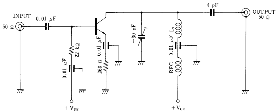
100 MHz G_{pe} NF 測定回路/TEST CIRCUIT
