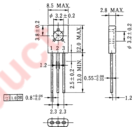
外形図 (単位: mm)
