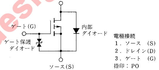
等価回路
