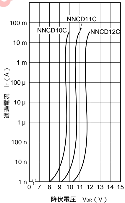
図3 . VBR-IT特性例 ( 2 )
