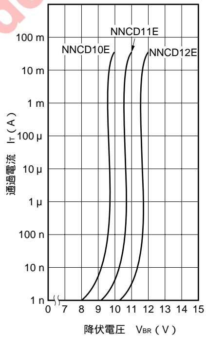
図3 . V BR -I T 特性例 ( 2 )
