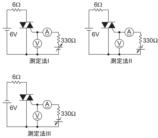
ゲートトリガ特性測定回路
