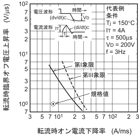
転流特性 ( T_j = 150^\circ\text{C} )
