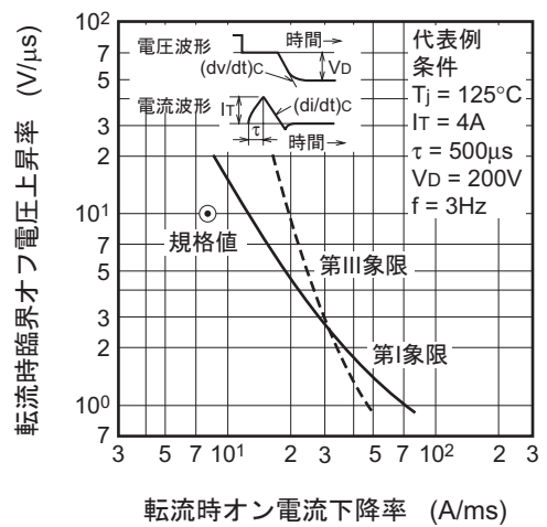
転流特性 (T j = 125°C)
