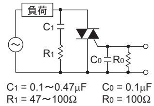
周辺回路定数の推奨値
