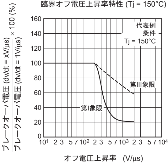
臨界オフ電圧上昇率特性 (T j = 150°C)
