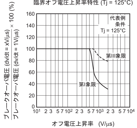
臨界オフ電圧上昇率特性 (T j = 125°C)
