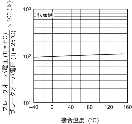
ブレイクオーバー電圧—接合温度
