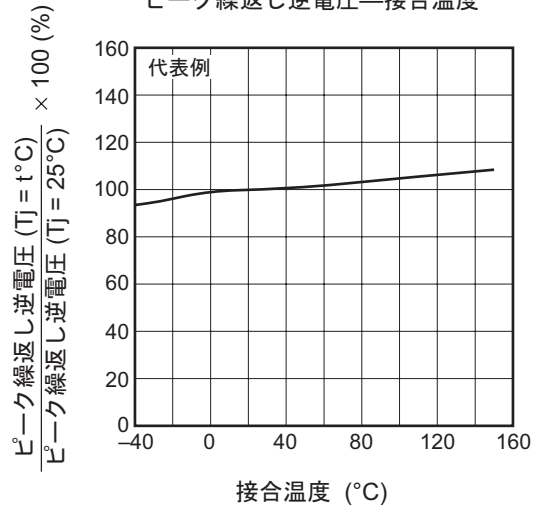
ピーク繰返し逆電圧—接合温度
