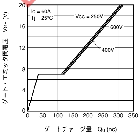
ゲート・エミッタ間電圧 - ゲートチャージ量特性 (代表例)
