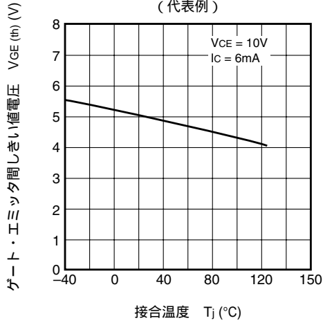
ゲート・エミッタ間しきい値電圧 - 接合温度特性 (代表例)
