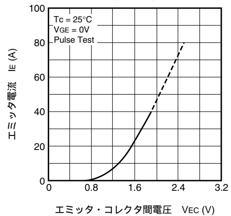
エミッタ電流 - エミッタ・コレクタ間電圧特性 (代表例)
