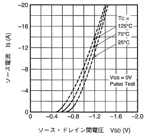
ソース電流— ソース・ドレイン間電圧特性 (代表例)
