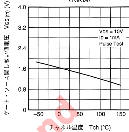
ゲート・ソース間しきい値電圧— チャンネル温度特性 (代表例)
