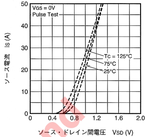
ソース電流ー ソース・ドレイン間電圧 (代表例)
