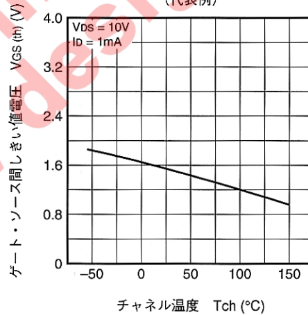
ゲート・ソース間しきい値電圧ー チャネル温度特性 (代表例)
