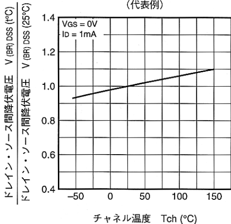
ドレイン・ソース間降伏電圧ー チャネル温度特性 (代表例)
