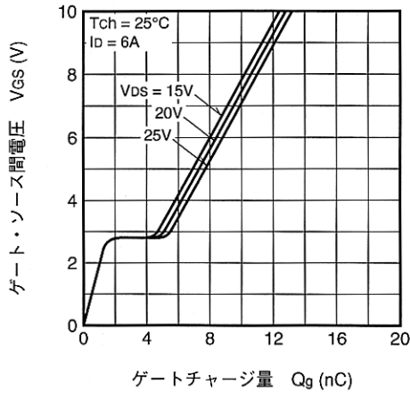
ゲート・ソース間電圧ー ゲートチャージ量特性 (代表例)
