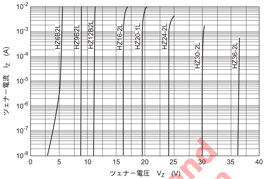
図1. ツェナー特性
