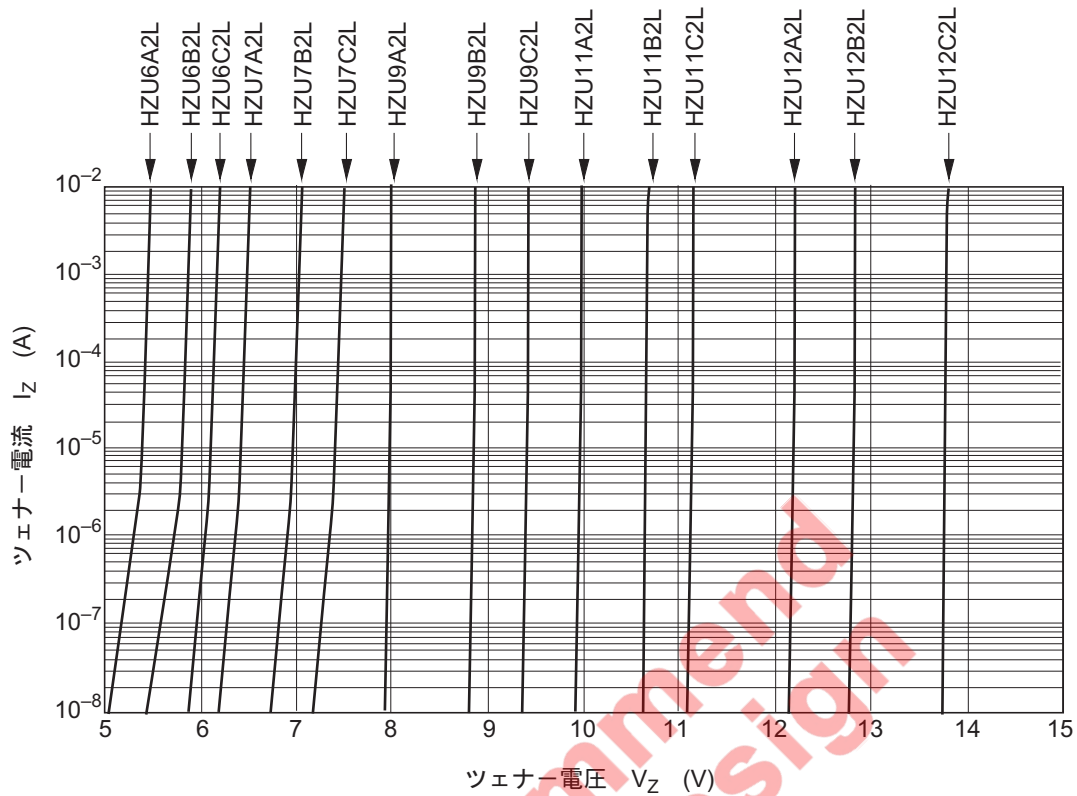
図1. ツェナー特性
