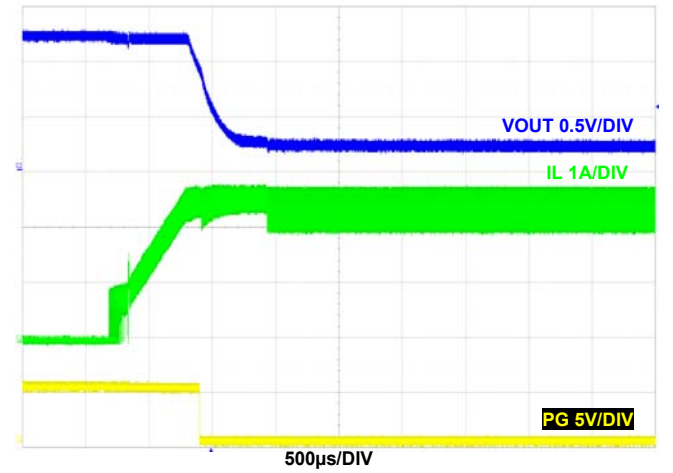
図 48. 過電流保護 F_{SW} = 2\text{MHz} 、 V_{IN} = 5\text{V} 、MODE = PWM、 T_A = +25^\circ\text{C}
