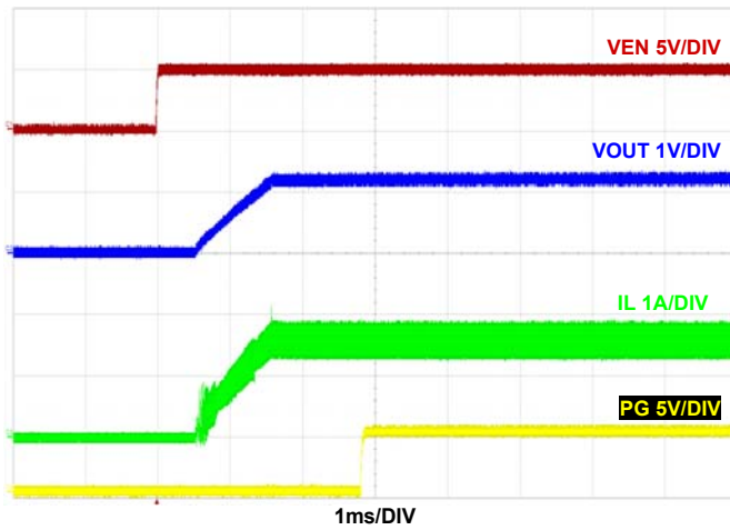
図 29. 1.5A 負荷時のスタートアップ F_{SW} = 2\text{MHz} , V_{IN} = 5\text{V} , \text{MODE} = \text{PWM} , T_A = +25^\circ\text{C}
