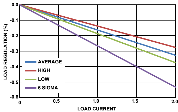
図 14. ロード・レギュレーション T_A = +105^\circ\text{C} , 5.5\text{V}_{IN} , 0.6\text{V}_{OUT} , 1\text{MHz}
