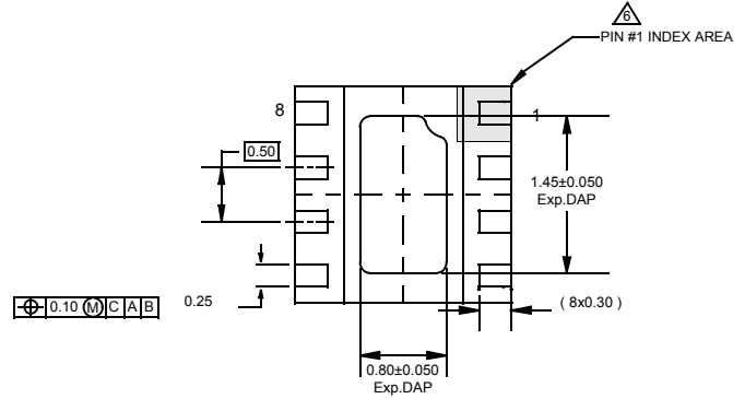
底面図
