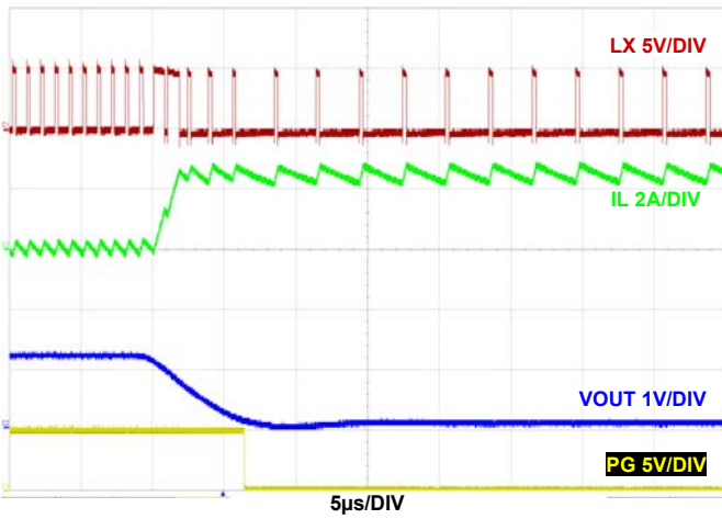
図 47. 出力短絡 F_{SW} = 2\text{MHz} 、 V_{IN} = 5\text{V} 、MODE = PFM、 T_A = +25^\circ\text{C}
