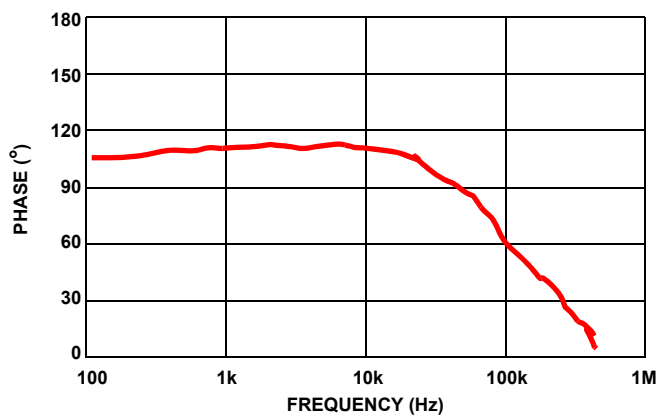
図 57. ループ・ゲインのシミュレーション結果
