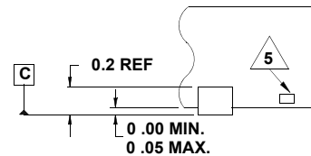
"X"の詳細
