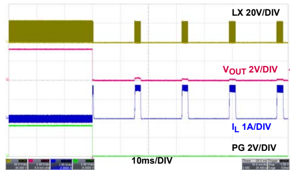
図 38. 過電流保護ヒックアップモード動作、PWM
