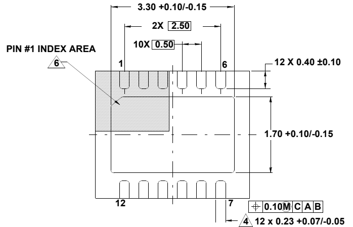
底面図
