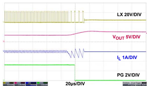
図 40. 逆電流保護動作、PWM
