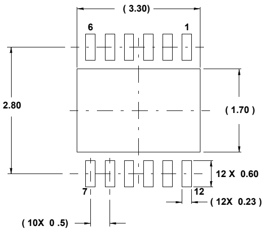
推奨ランドパターン例
