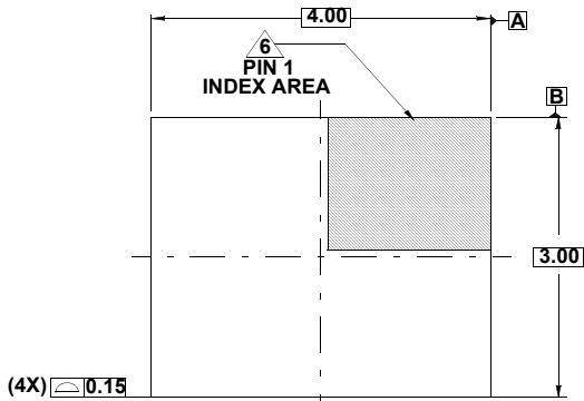
上面図
