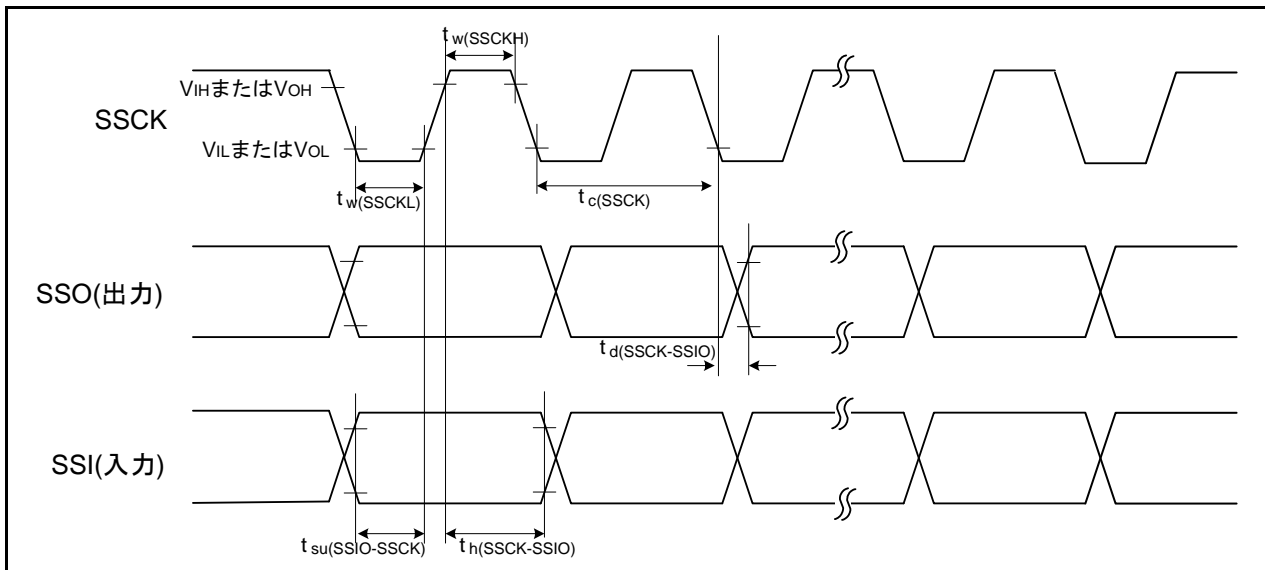
図 5.61 シリアルバスインタフェースの入出力タイミング図 (クロック同期式通信モード)
