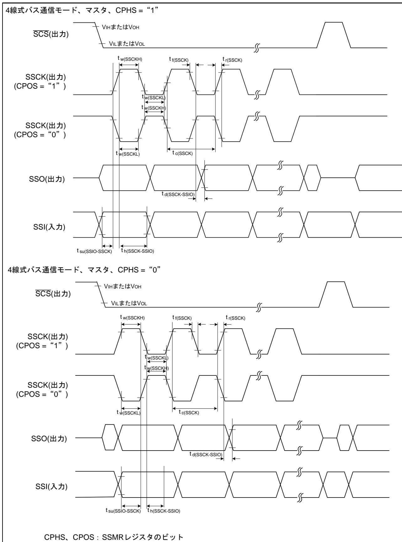
図 5.28 シリアルバスインタフェースの入出力タイミング (マスタ)
