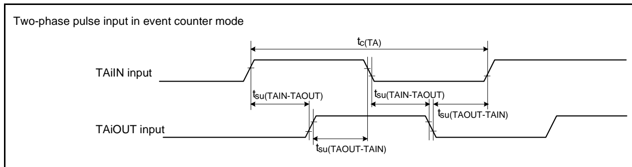
図 5.22 タイマA入力(イベントカウンタモードの二相パルス入力)
