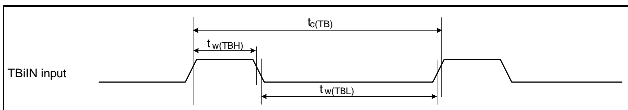
図 5.54 タイマB入力
