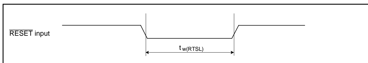
図 5.19 リセット入力 ( \overline{RESET} 入力)
