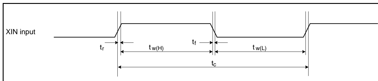
図 5.20 外部クロック入力 (XIN入力)
