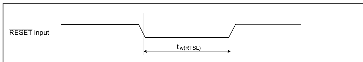
図 5.37 リセット入力 ( \overline{RESET} 入力)
