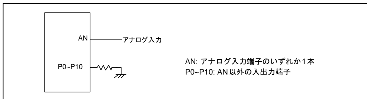
図 5.34 A/D精度測定回路
