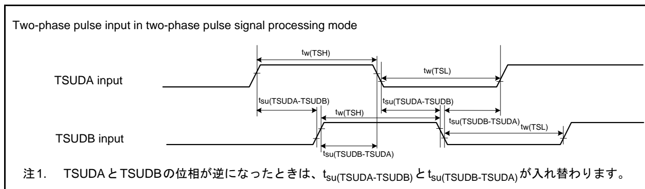
図 5.42 タイマS入力(二相パルス信号処理モードの二相パルス入力)
