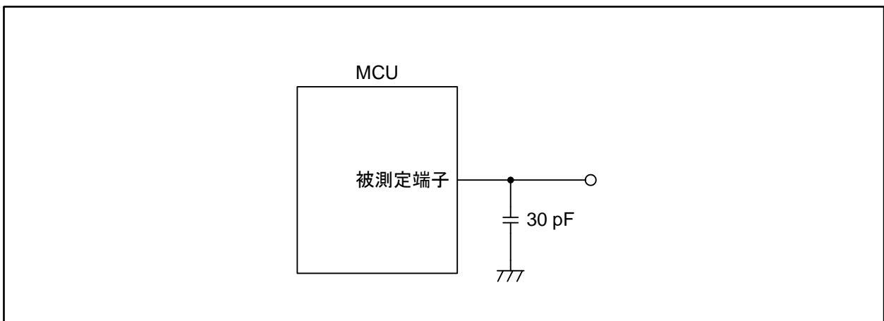
図 5.49 スイッチング特性の測定回路
