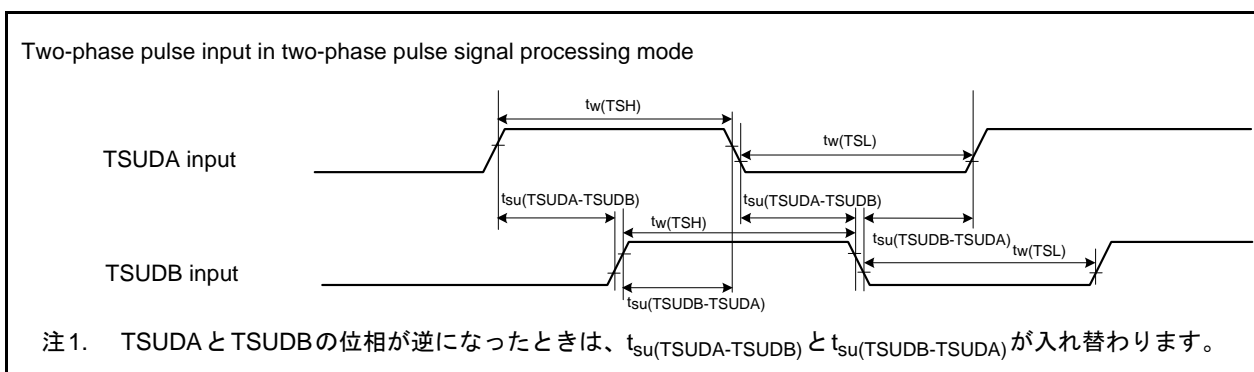
図 5.24 タイマS入力(二相パルス信号処理モードの二相パルス入力)
