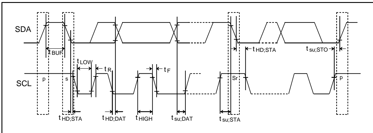
図 5.14 マルチマスタ I 2 C-bus
