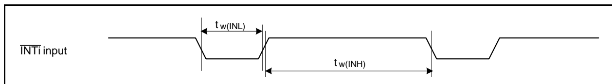
図 5.57 外部割り込み \overline{INTi} 入力
