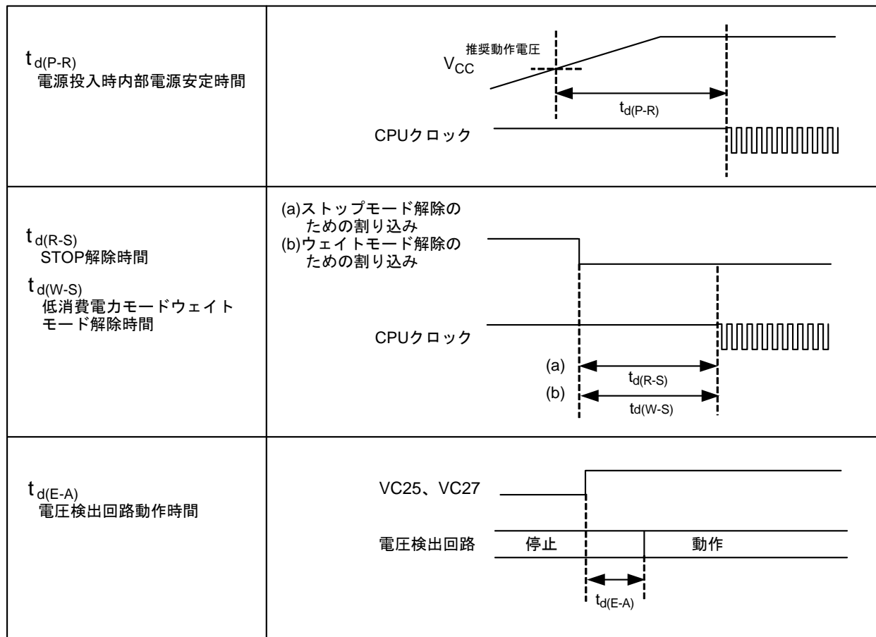
図 5.36 電源回路のタイミング図
