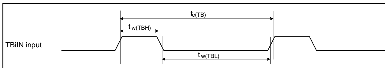
図 5.23 タイマB入力
