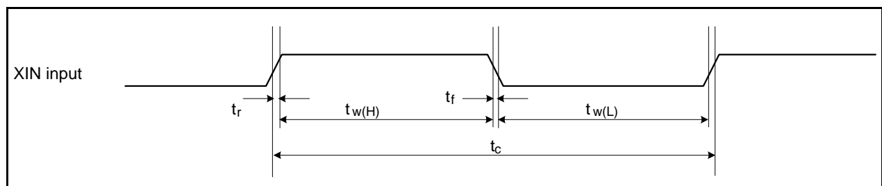
図 5.51 外部クロック入力 (XIN入力)
