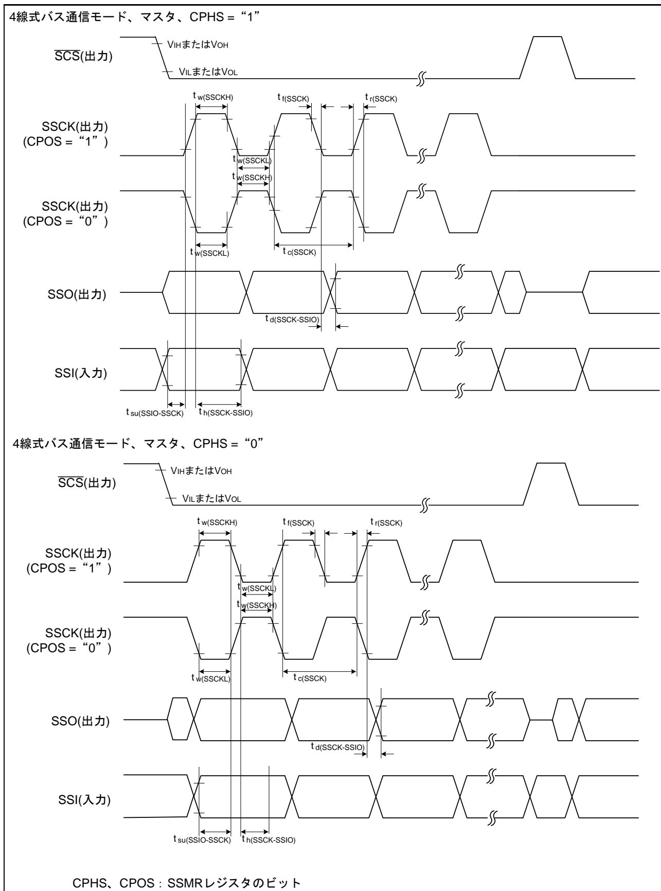
図 5.15 シリアルバスインタフェースの入出力タイミング (マスタ)
