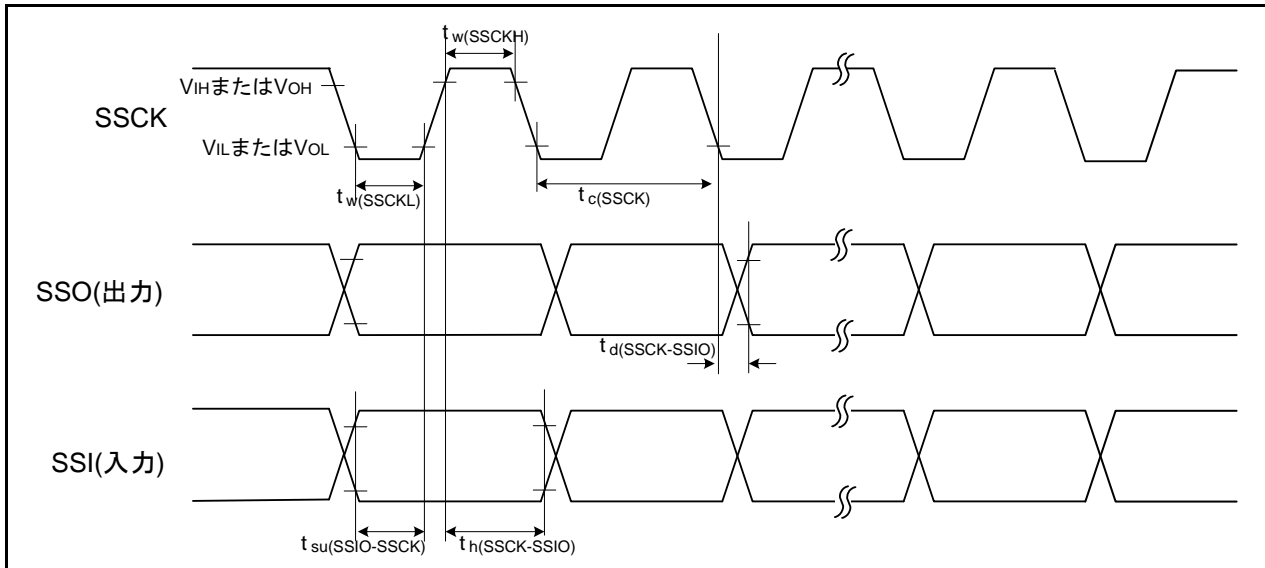
図 5.17 シリアルバスインタフェースの入出力タイミング図 (クロック同期式通信モード)
