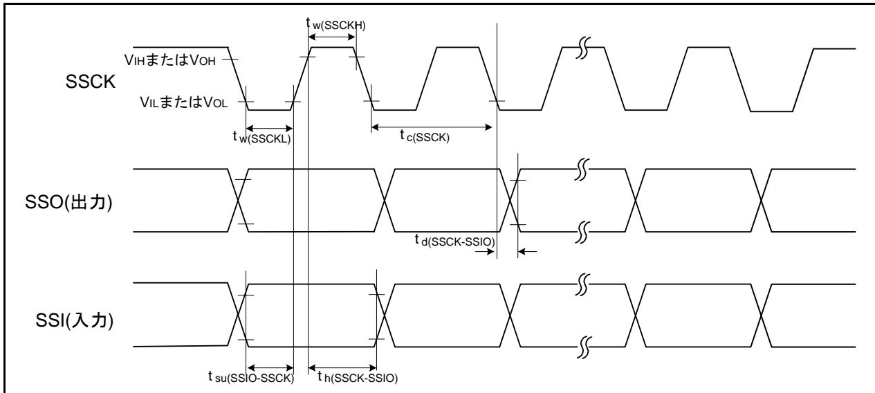
図 5.30 シリアルバスインタフェースの入出力タイミング図 (クロック同期式通信モード)
