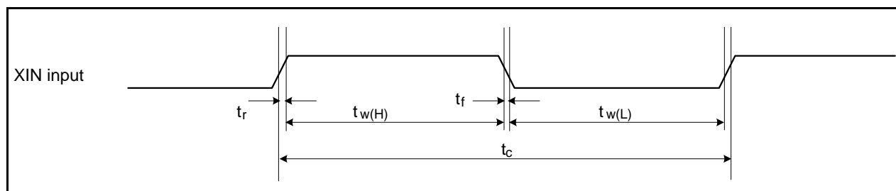
図 5.38 外部クロック入力 (XIN入力)
