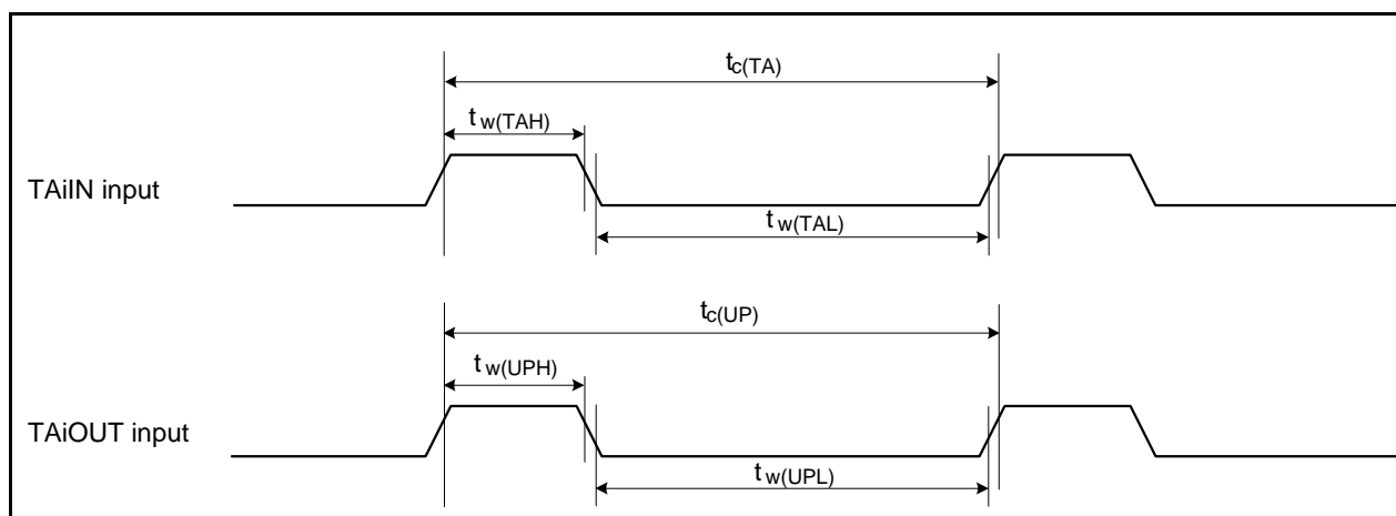
図 5.21 タイマA入力
