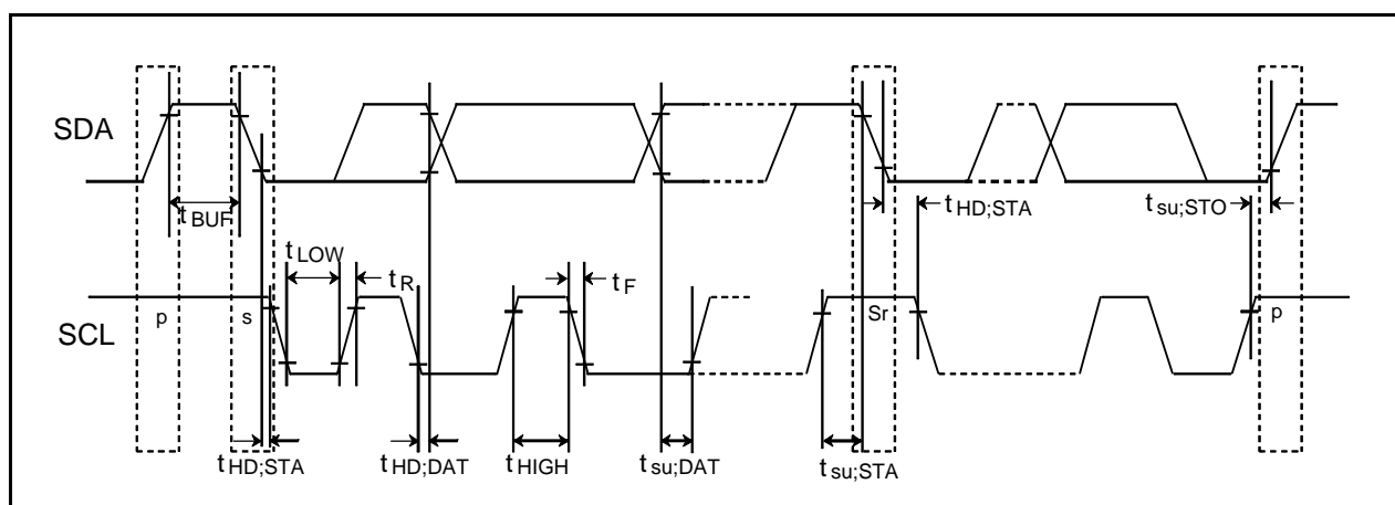
図 5.58 マルチマスタ I 2 C-bus
