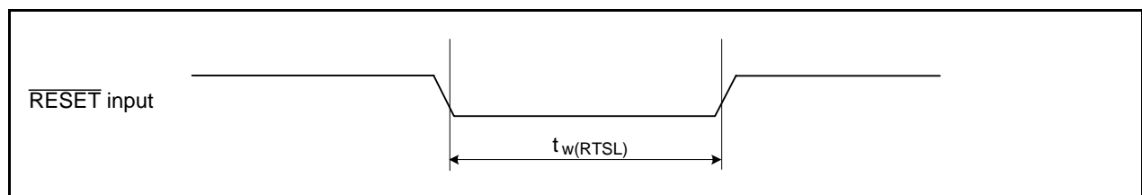
図 5.50 リセット入力 ( \overline{RESET} 入力)
