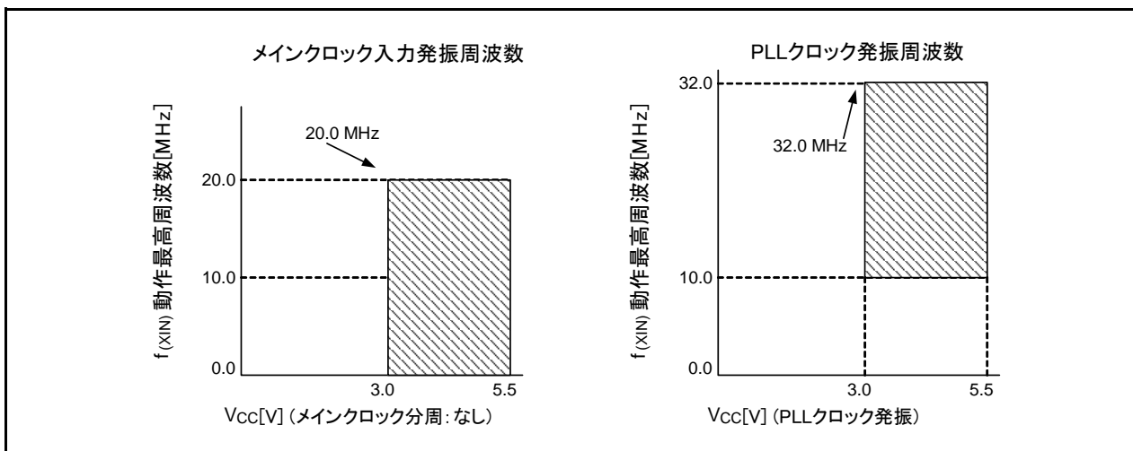
図 5.32 メインクロック発振周波数、PLLクロック発振周波数
