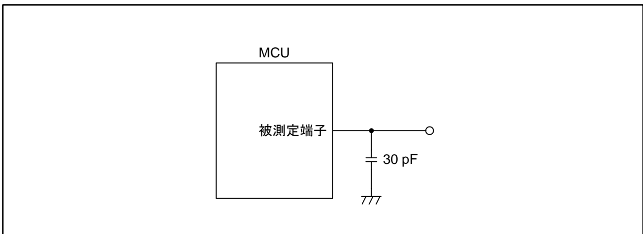
図 5.31 スイッチング特性の測定回路
