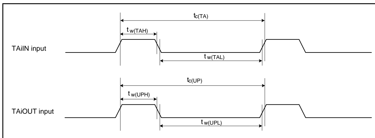
図 5.52 タイマA入力
