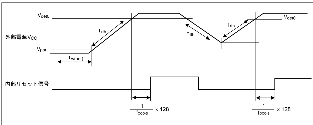
図5.35 パワーオンリセット回路の電气的特性
