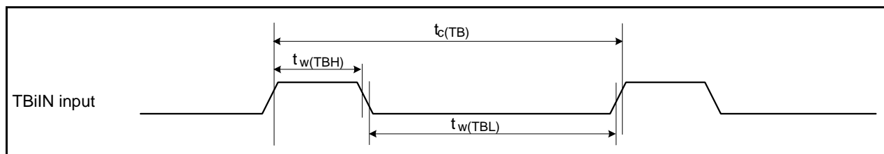
図 5.41 タイマB入力
