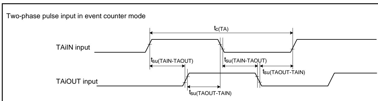
図 5.53 タイマA入力(イベントカウンタモードの二相パルス入力)
