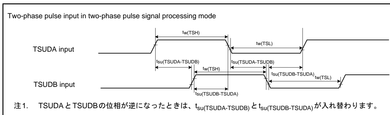
図 5.55 タイマS入力(二相パルス信号処理モードの二相パルス入力)
