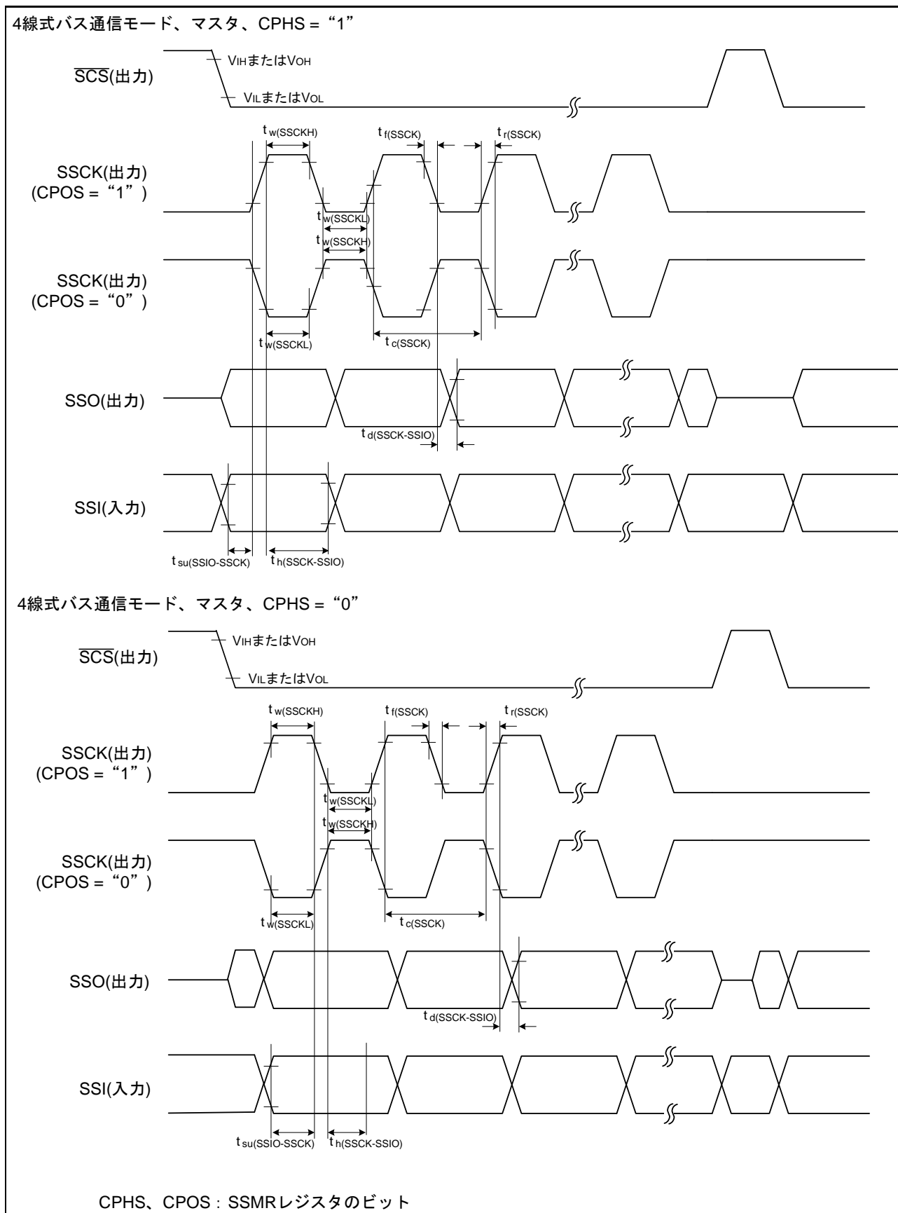
図 5.59 シリアルバスインタフェースの入出力タイミング (マスタ)
