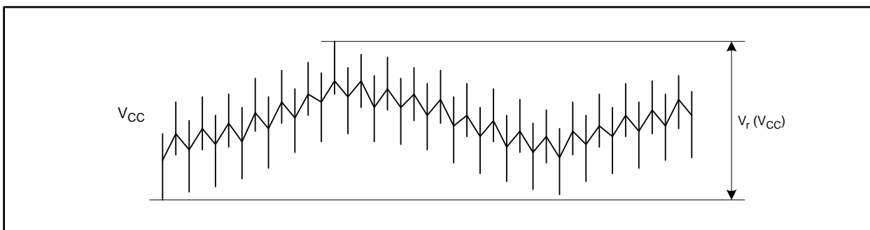
図 5.33 電源リップル波形
