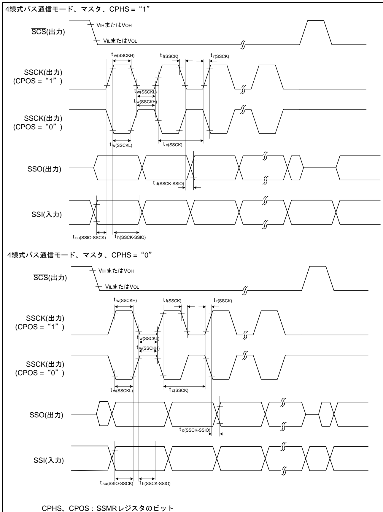
図 5.46 シリアルバスインタフェースの入出力タイミング (マスタ)
