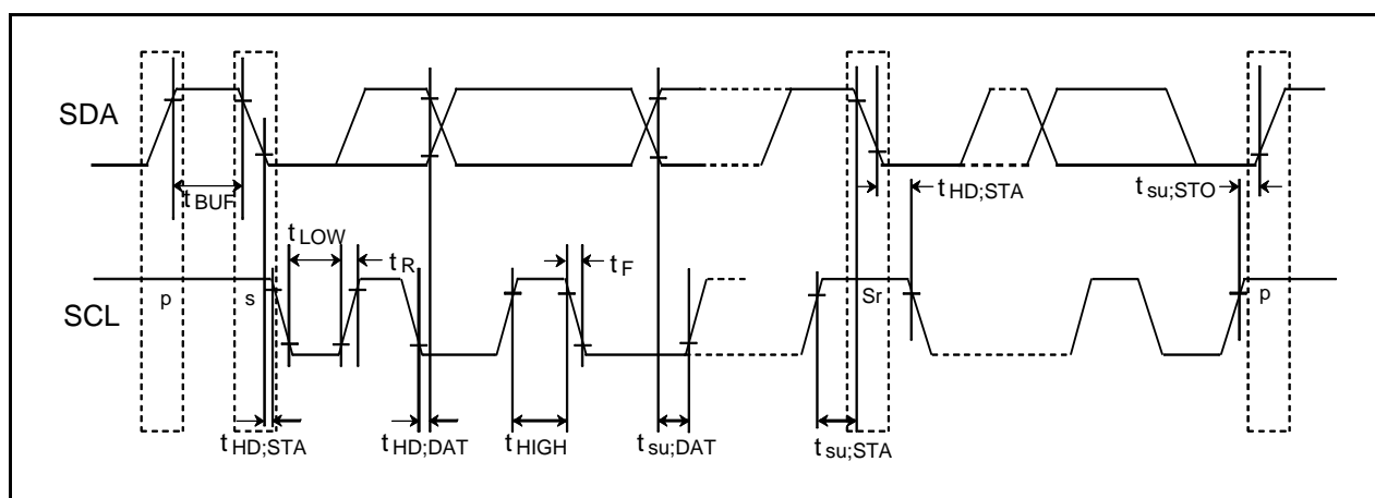
図 5.45 マルチマスタ I 2 C-bus
