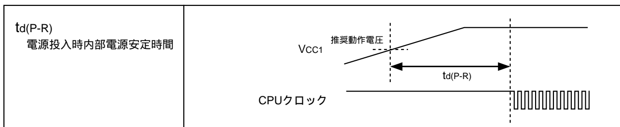
図5.11 電源回路のタイミング図
