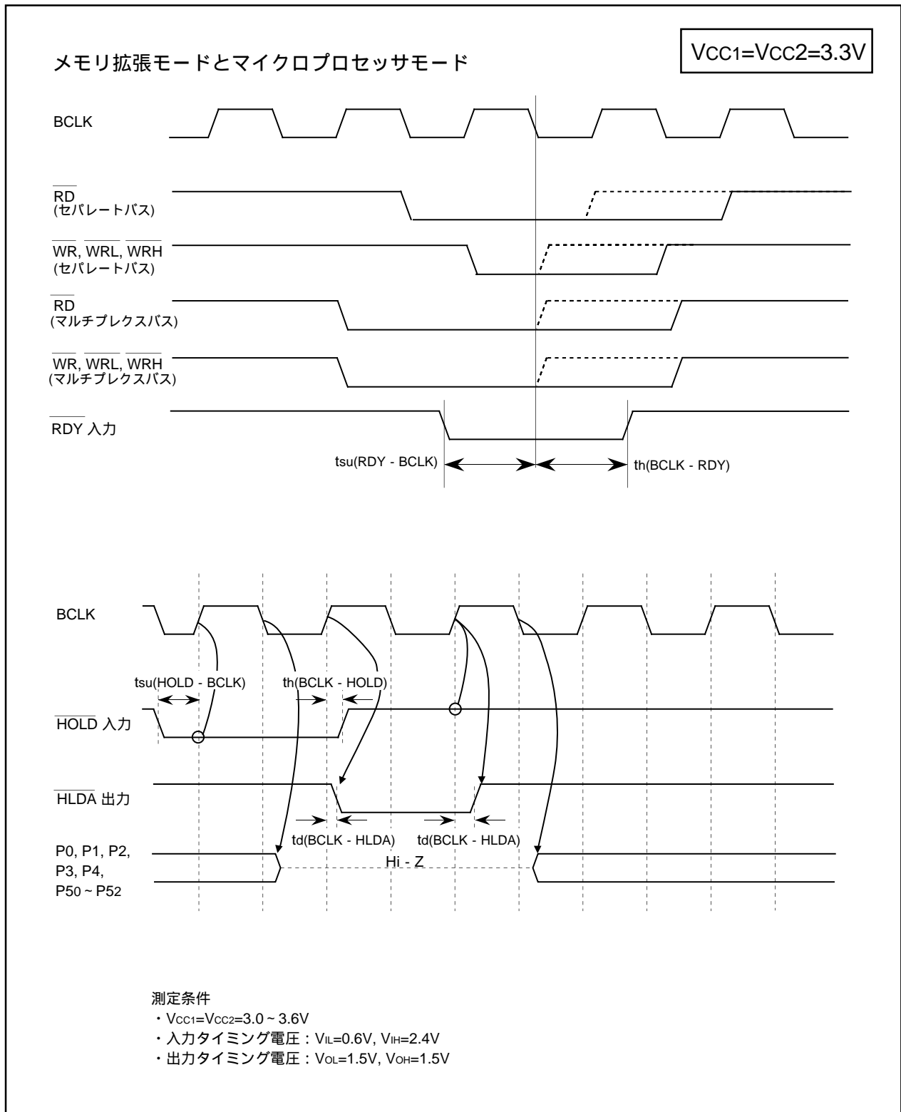
図5.10 VCC1=VCC2=3.3V時のタイミング図(4)
