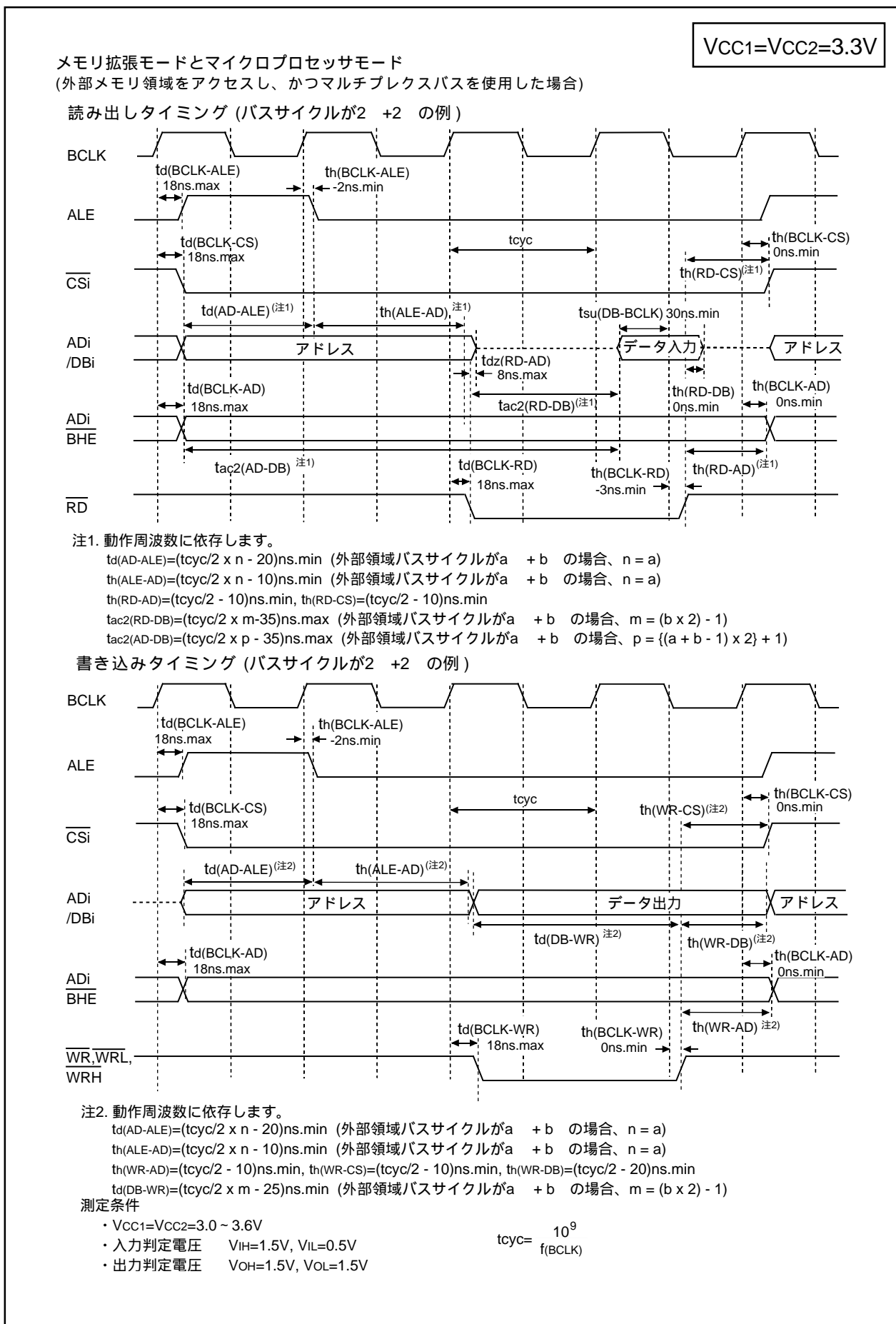
図5.8 VCC1=VCC2=3.3V時のタイミング図(2)
