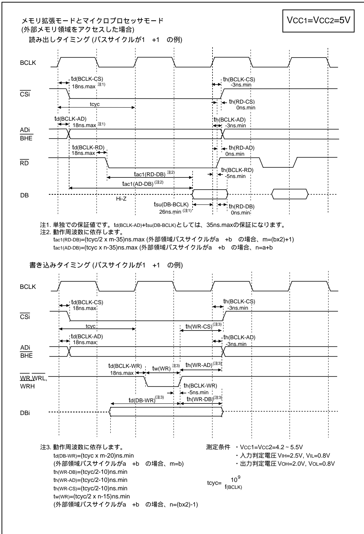
図5.3 Vcc1=Vcc2=5V時のタイミング図(1)
