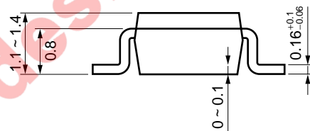
(5ピン・ミニモールド)
