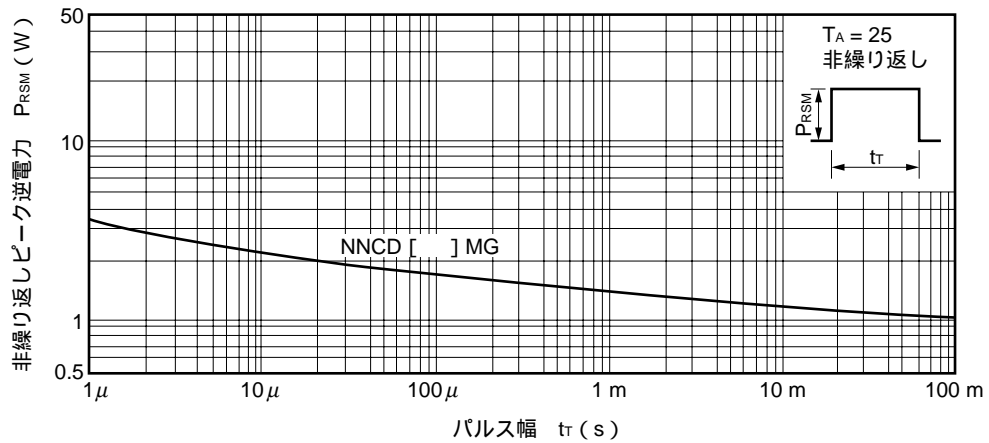
図5. サージ逆電力定格
