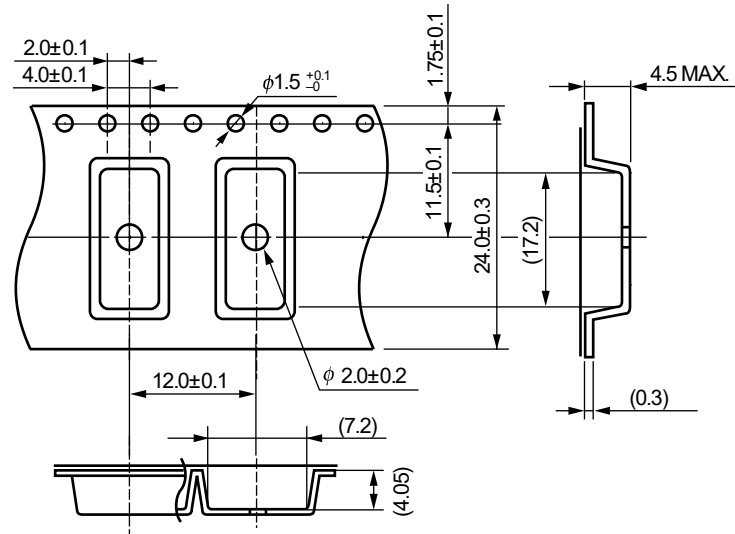
外形および寸法 (テープ)
