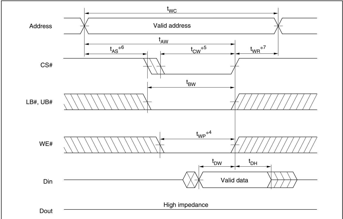
ライトタイミング波形 (2) (CS# Clock, OE# = V IH )
