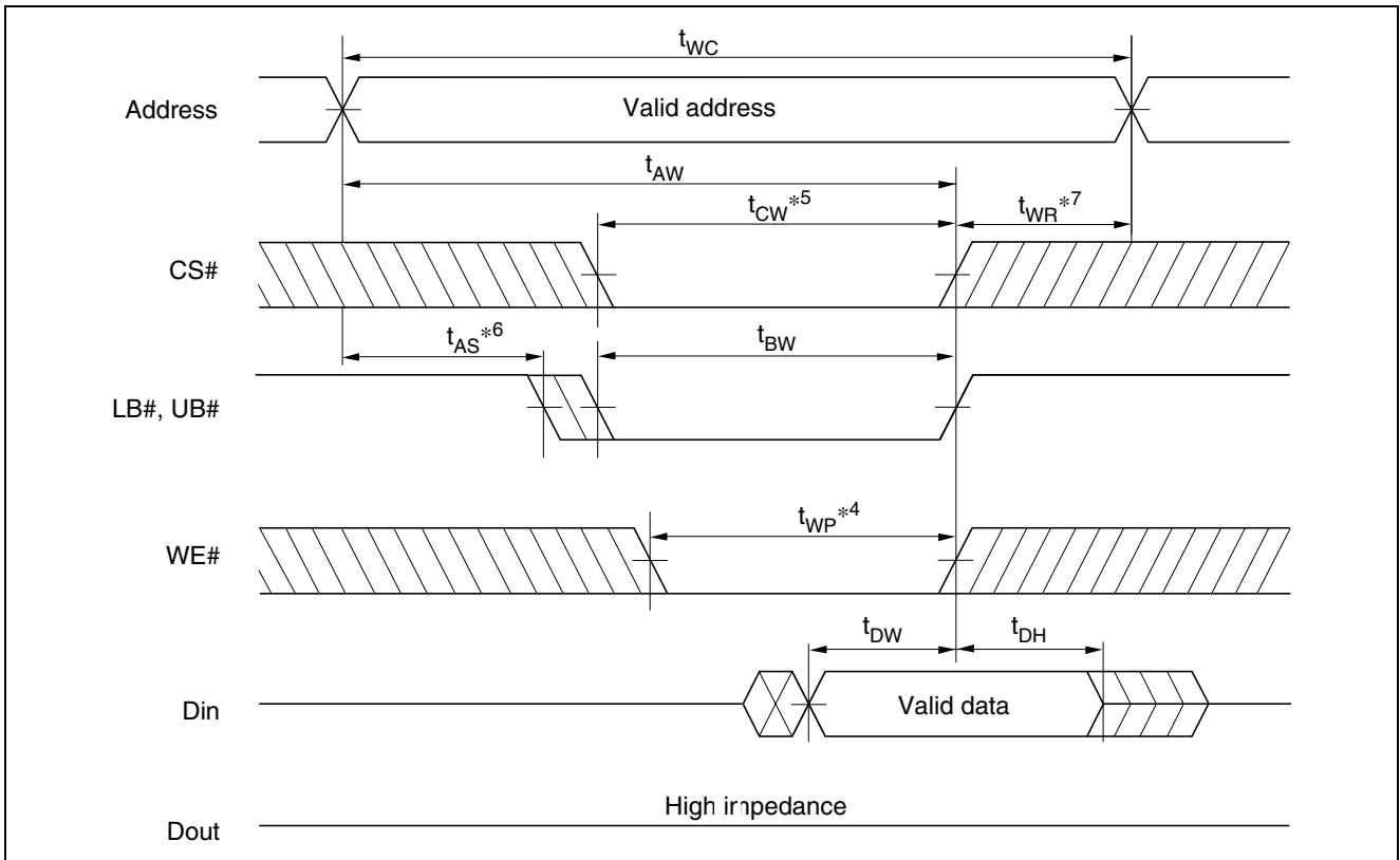
ライトタイミング波形 (3) (LB#, UB# Clock, OE# = V IH )
