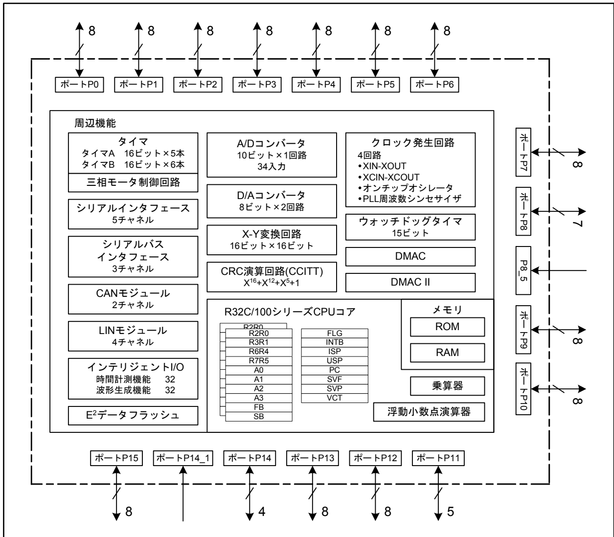
図 1.2 R32C/156グループのブロック図
