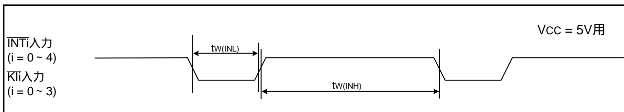
図5.11 Vcc = 5V時の外部割り込み \overline{\text{INT}}_i およびキー入力割り込み \overline{\text{Kli}} 入力タイミング
