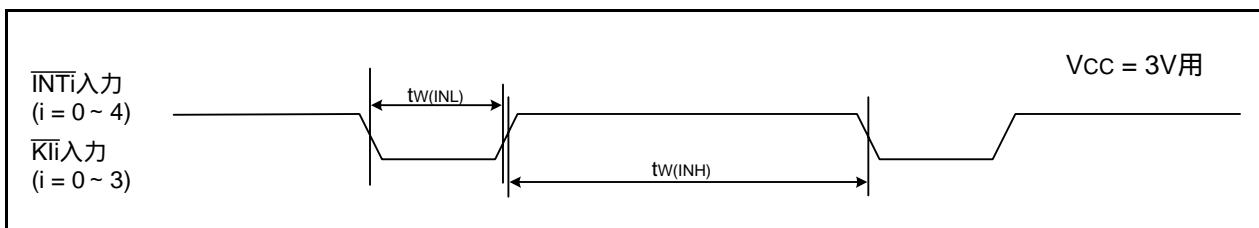
図5.16 Vcc = 3V時の外部割り込みINTiおよびキー入力割り込みKli入力タイミング
