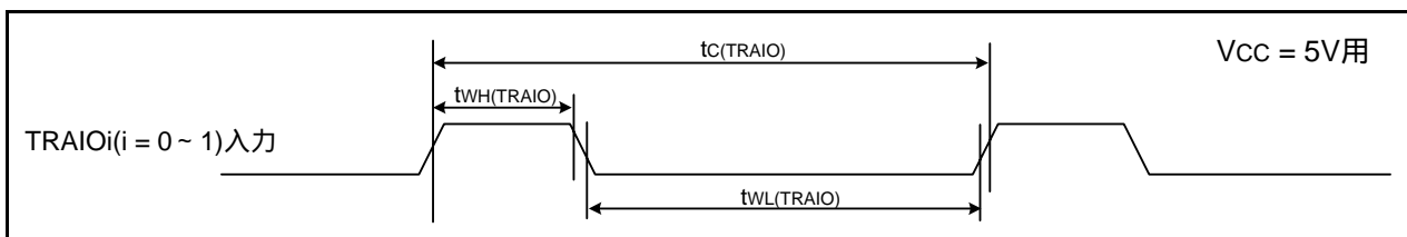
図5.8 VCC = 5V時のTRAI0i(0, 1)入力タイミング
