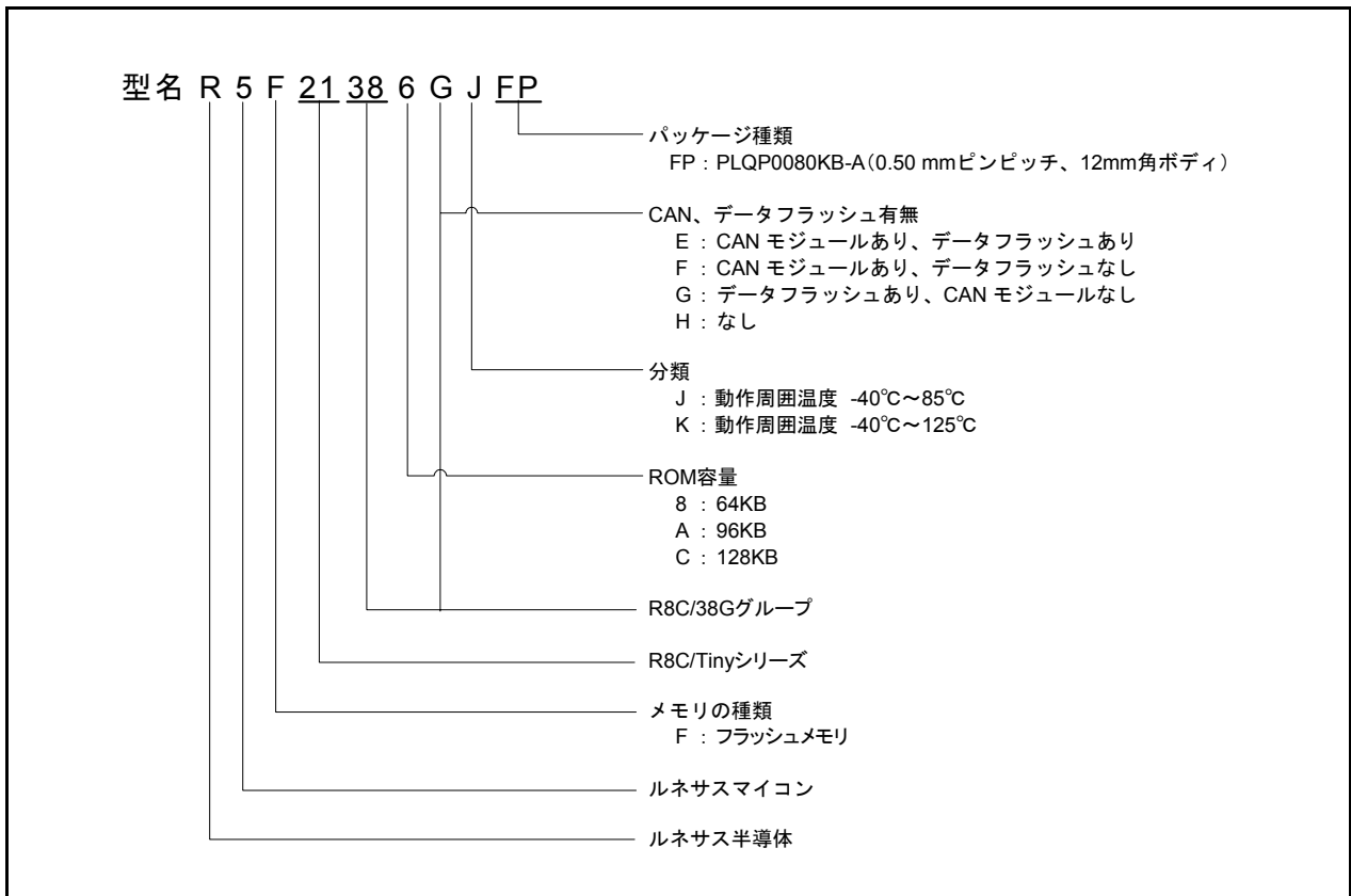
図 1.3 R8C/38G グループの型名とメモリサイズ・パッケージ
