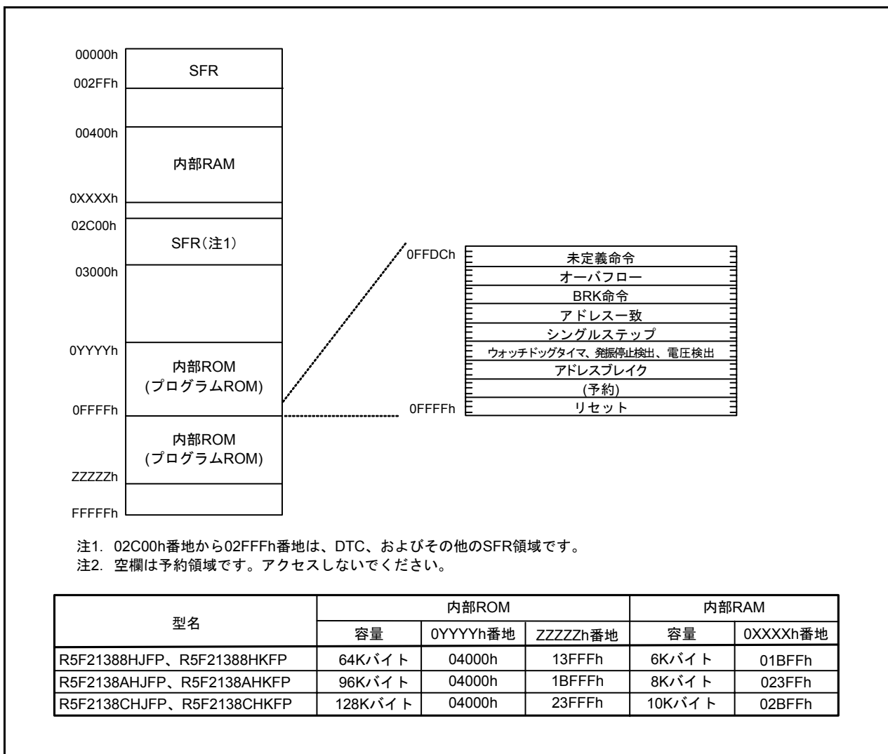
図3.4 R8C/38Hグループのメモリ配置図
