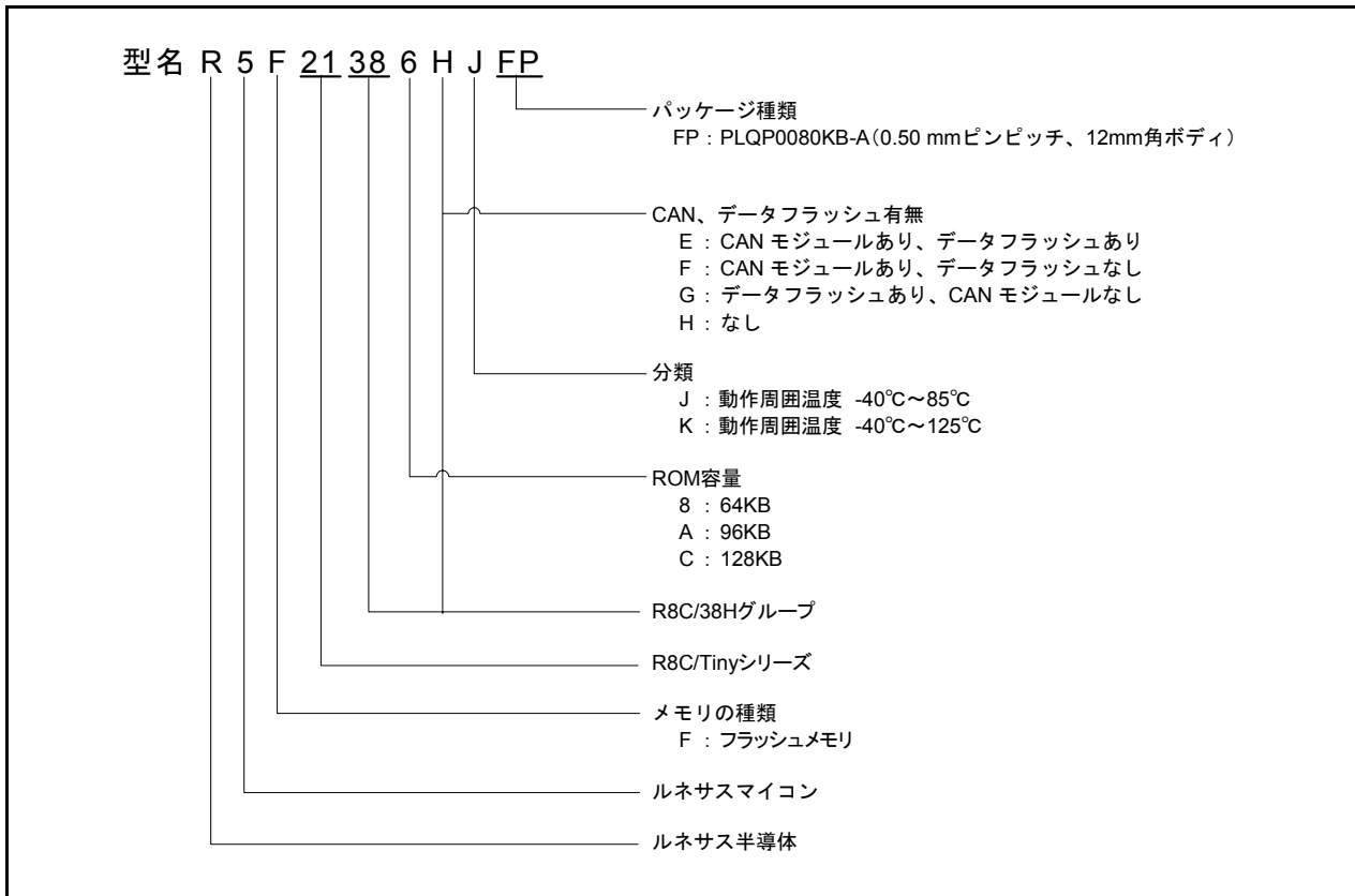
図 1.4 R8C/38Hグループの型名とメモリサイズ・パッケージ
