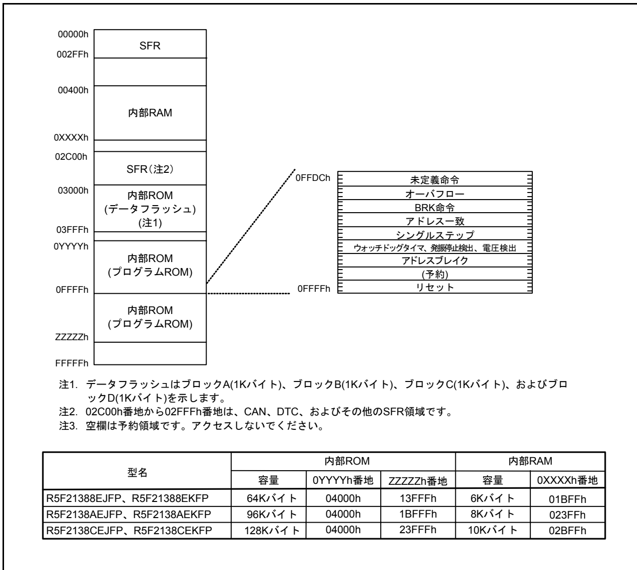
図3.1 R8C/38Eグループのメモリ配置図
