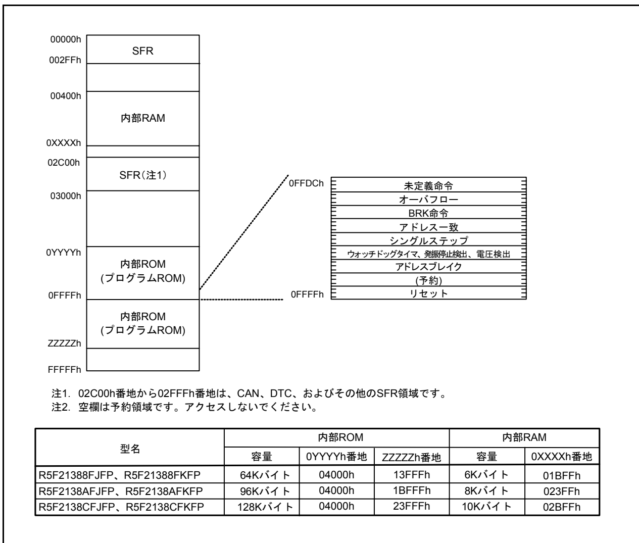
図3.2 R8C/38Fグループのメモリ配置図
