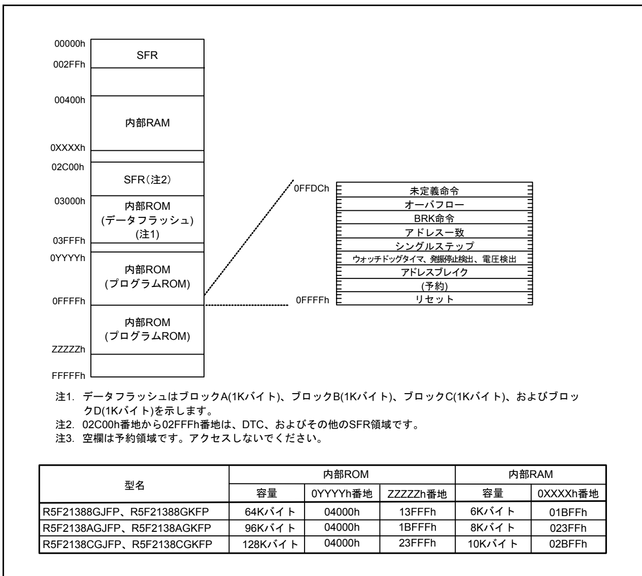
図3.3 R8C/38Gグループのメモリ配置図
