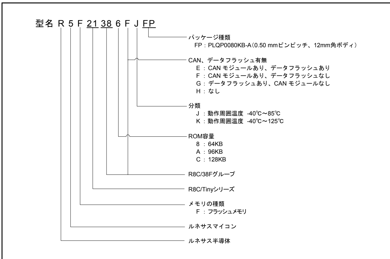
図 1.2 R8C/38F グループの型名とメモリサイズ・パッケージ
