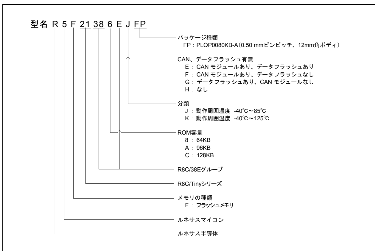
図 1.1 R8C/38Eグループの型名とメモリサイズ・パッケージ
