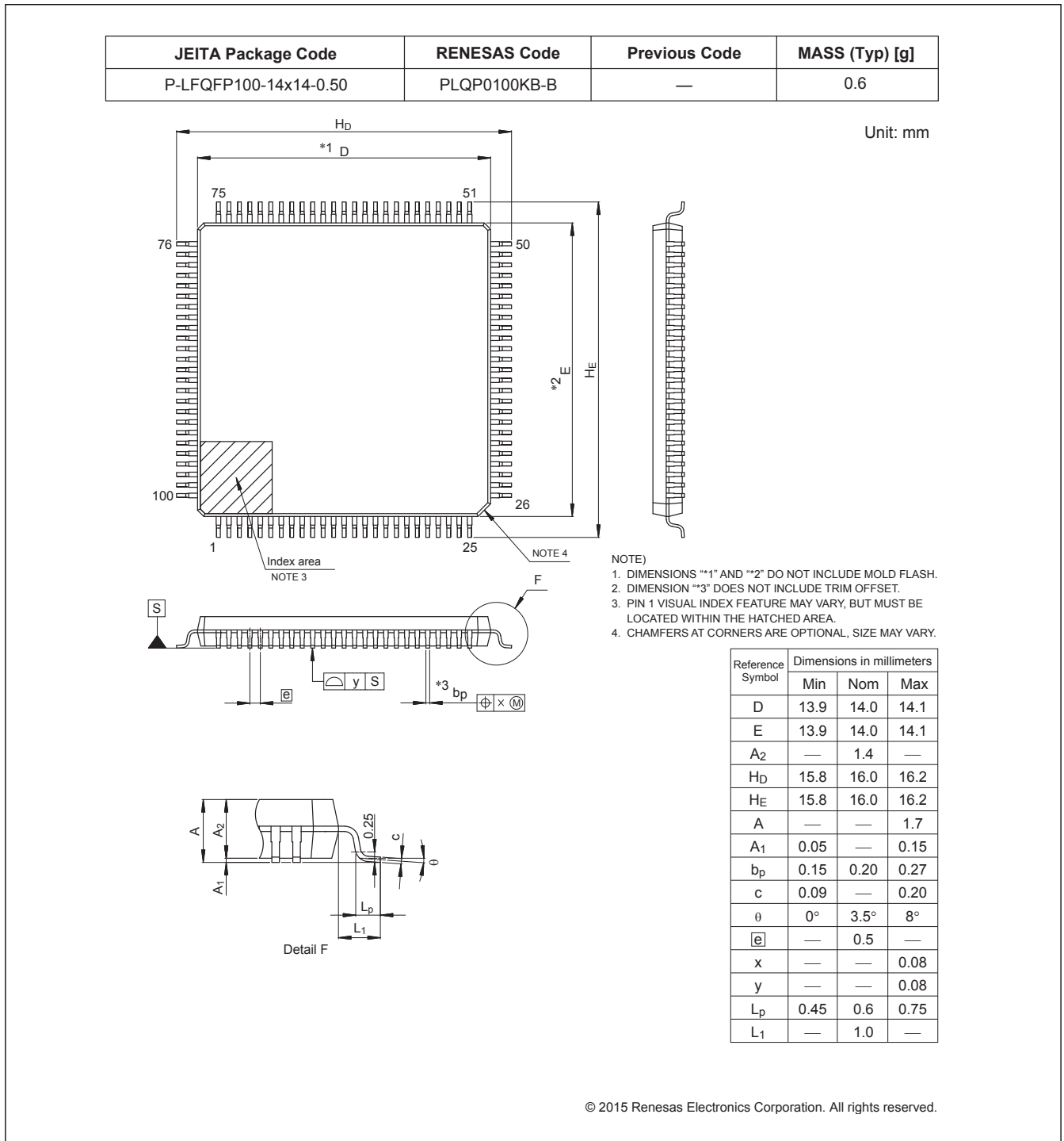
図 2.1 LQFP 100 ピン
