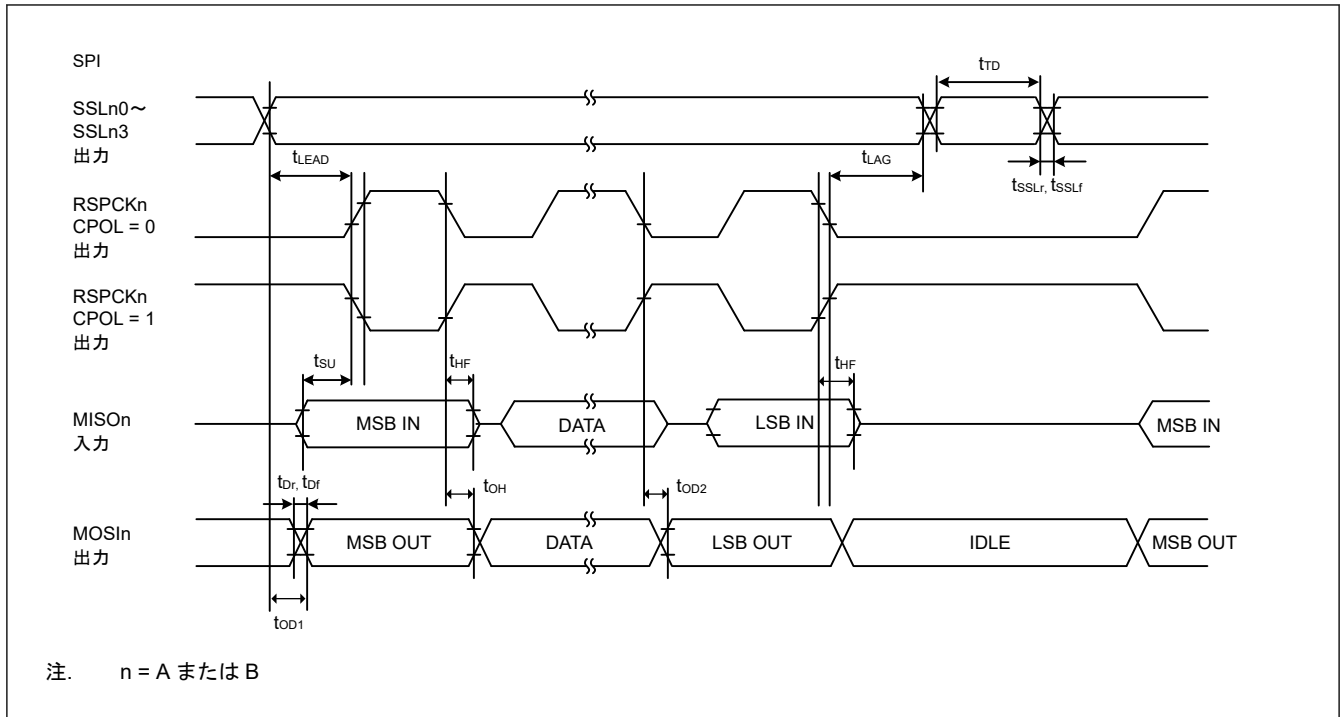
図 2.35 CPHA = 0 の場合、および PCLKA/2 にビットレートが設定されている場合におけるマスタの SPI タイミング
