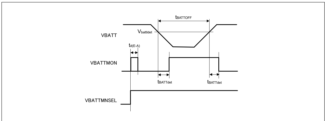
図 2.65 バッテリバックアップ機能特性
