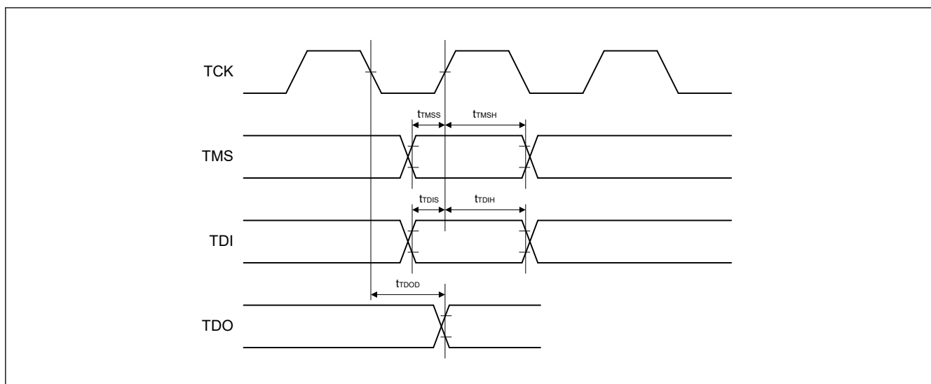
図 2.68 バウンダリスキャン入出力タイミング
