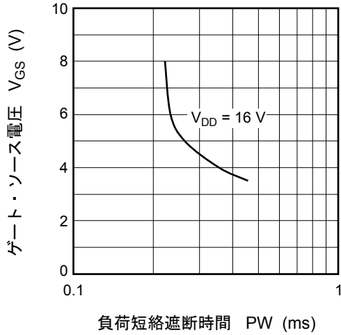
ゲート・ソース電圧対 負荷短絡遮断時間特性
