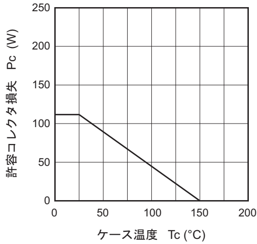
許容コレクタ損失の ケース温度による変化
