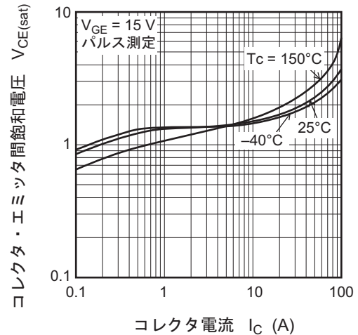
コレクタ・エミッタ間飽和電圧対 コレクタ電流特性
