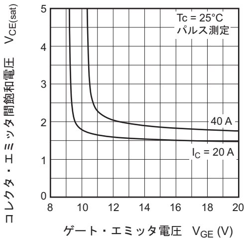
コレクタ・エミッタ間飽和電圧対 ゲート・エミッタ電圧特性
