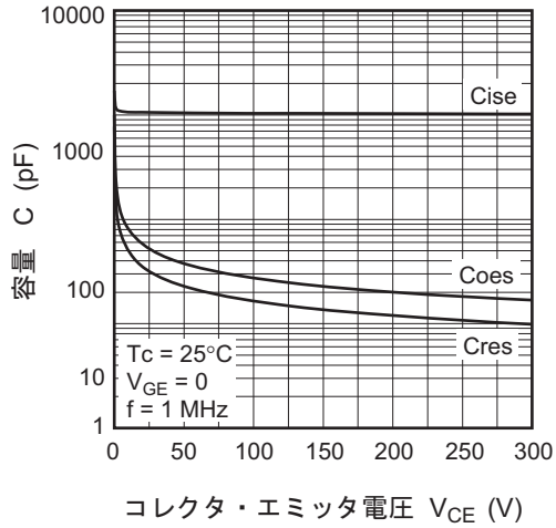
容量対コレクタ・エミッタ電圧特性
