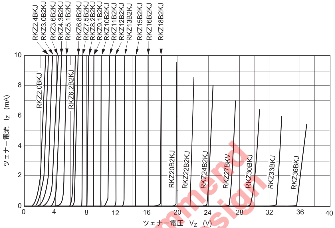
図1. ツェナー特性
