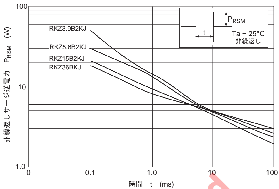
図4. サージ逆電力特性 (参考データ)
