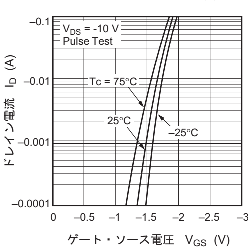
ソース接地伝達静特性 (2)
