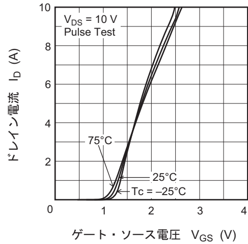
ソース接地伝達静特性 (1)
