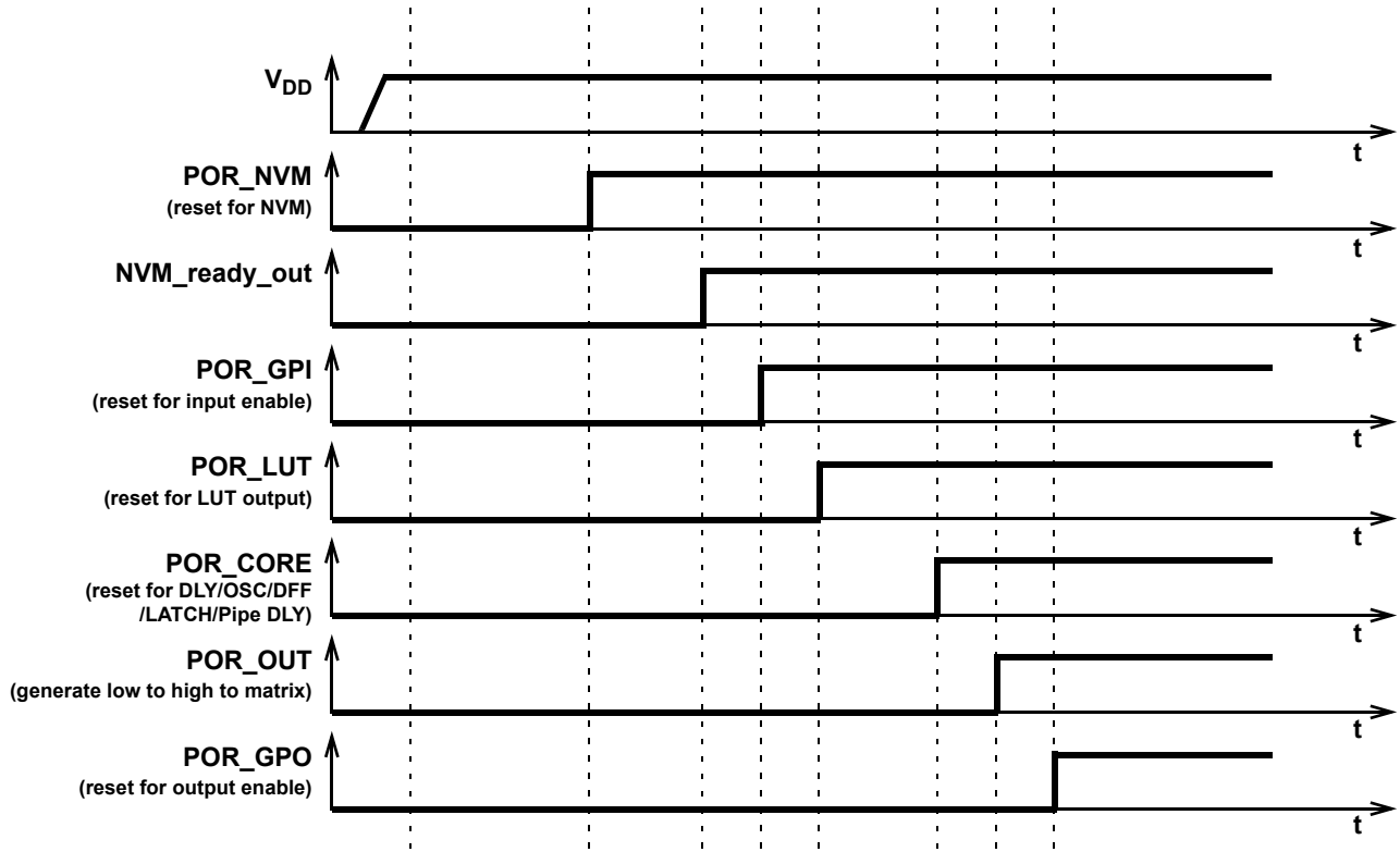
Figure 84. POR Sequence
