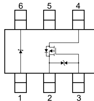
端子接続図 (Top View)
