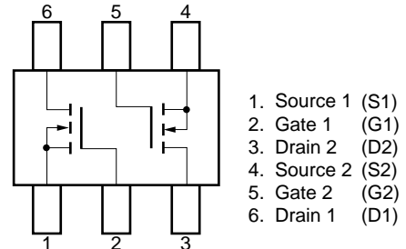
端子接続図
