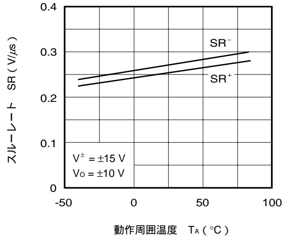
SR - T_A 特性
