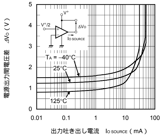
\Delta V_O - I_{O \text{ SOURCE}} 特性
