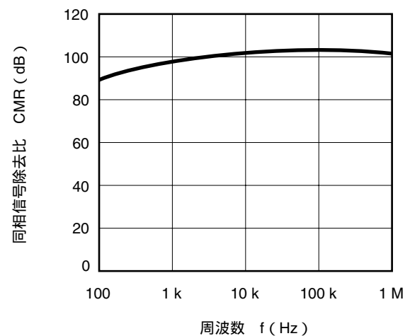
CMR - f 特性
