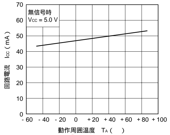
回路電流 vs. 動作周囲温度
