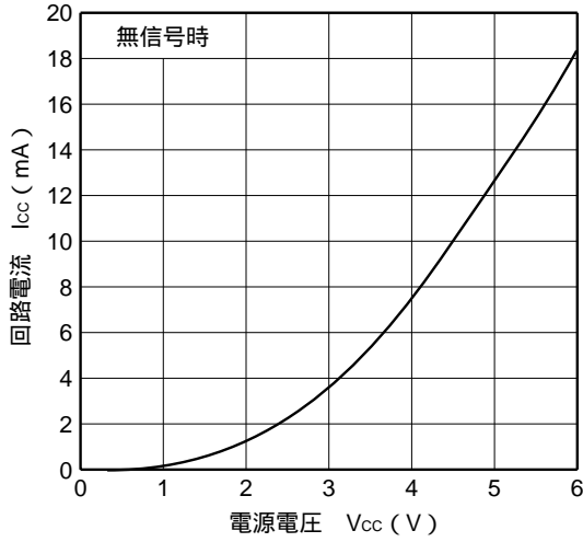
回路電流 vs. 電源電圧
