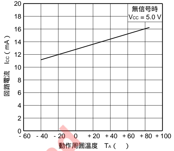
回路電流 vs. 動作周囲温度
