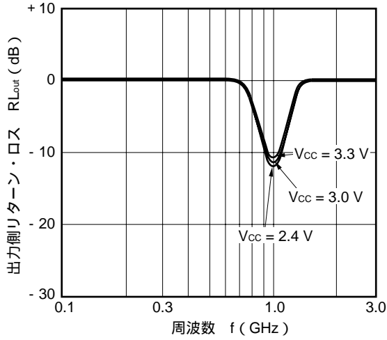
出力側リターン・ロス vs. 周波数
