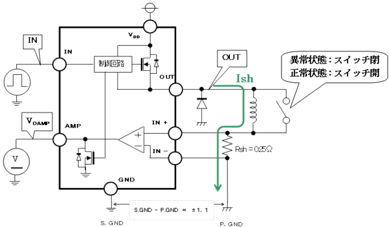
タイミングチャート測定回路
