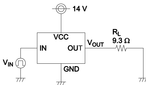
スイッチング測定回路
