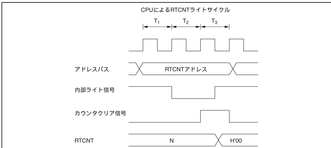
図 7.20 RTCNT のライトとクリアの競合
