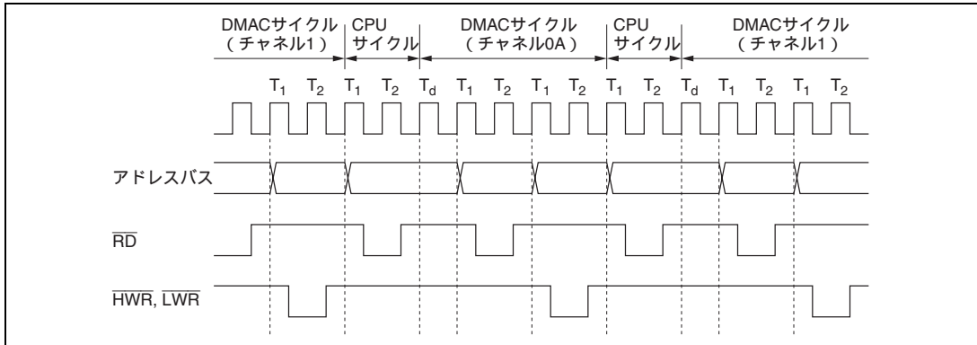
図 8.19 複数チャンネルの動作タイミング
