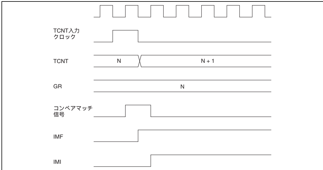
図 10.57 コンペアマッチ時の IMFA、IMFB フラグのセットタイミング
