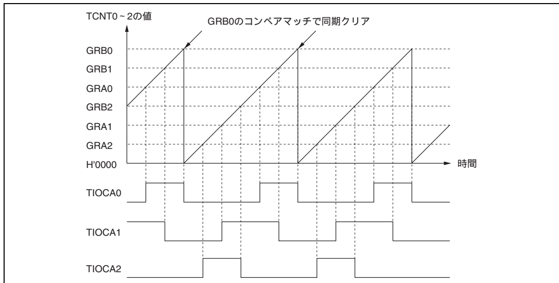
図 10.27 同期動作例
