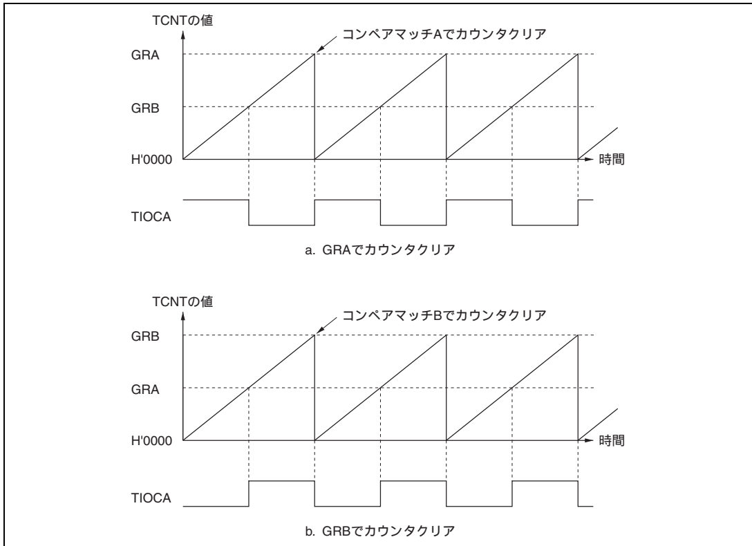
図 10.29 PWM モードの動作例 (1)
