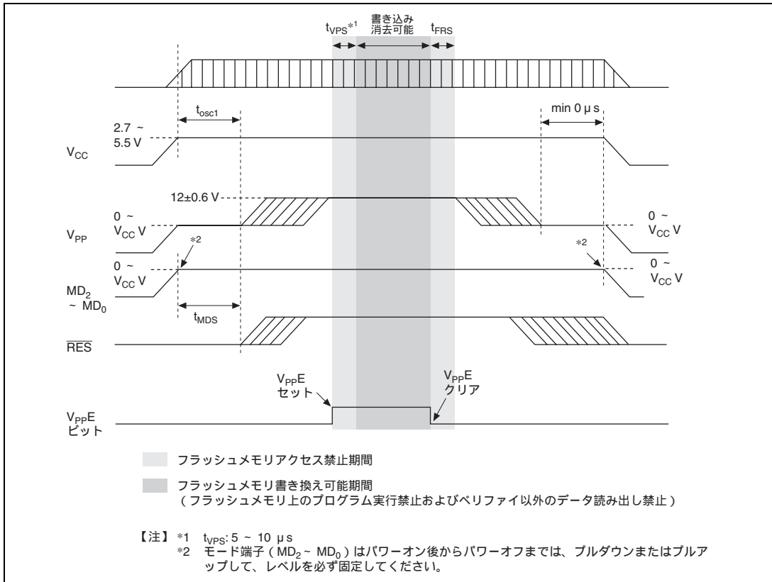
図 19.23 電源投入/切断タイミング (ユーザプログラムモード)
