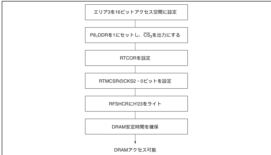
図 7.8 2WE 方式 1M ビット DRAM の設定順序 (1M バイトモード)
