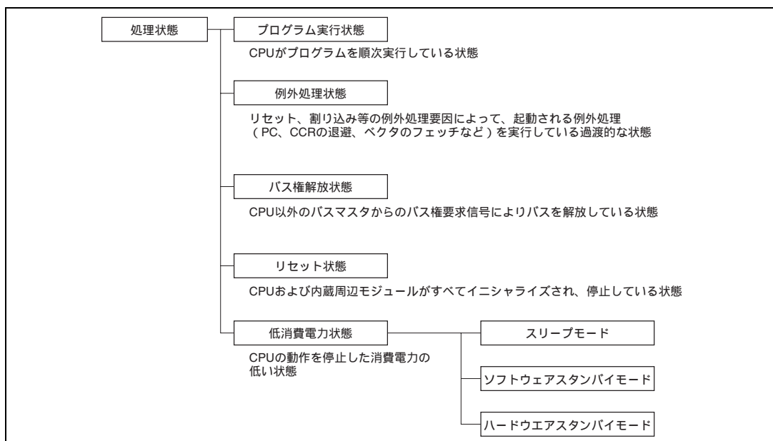
図 2.11 処理状態の分類
