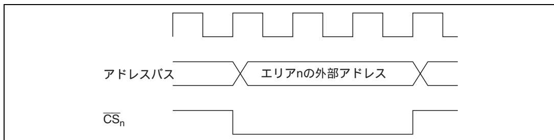
図 6.3 \overline{CS}_n 信号の出力タイミング ( n=7\sim 0 )
