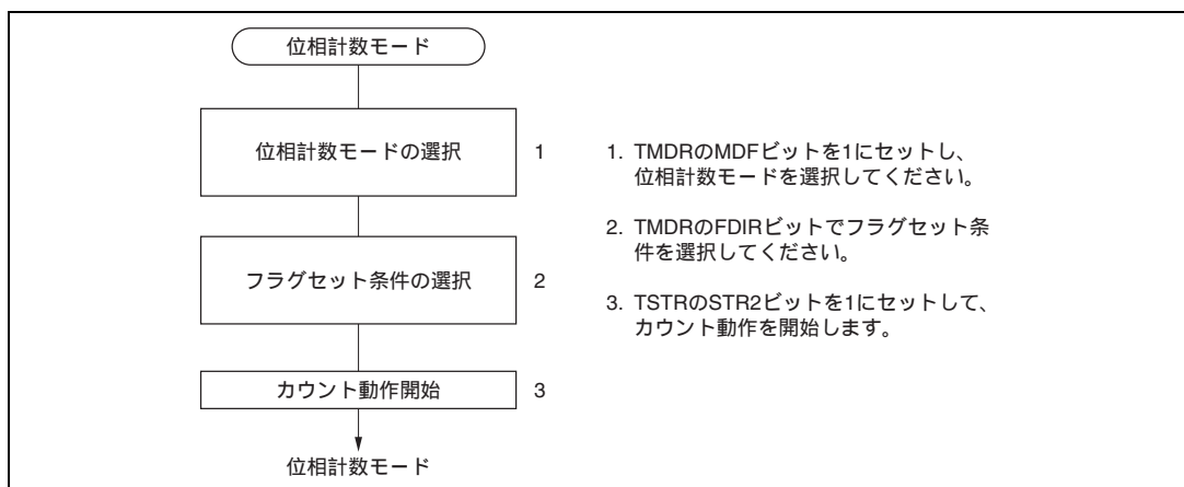
図 10.43 位相計数モードの設定手順例
