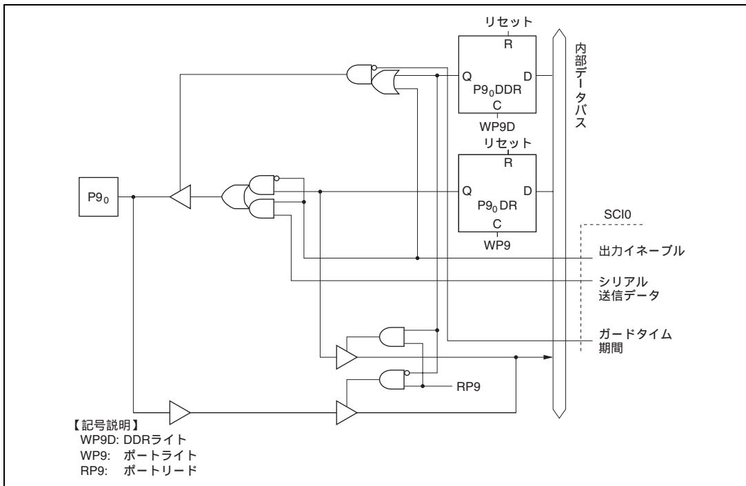
図C.9 (a) ポート9ブロック図 (P9 0 端子)
