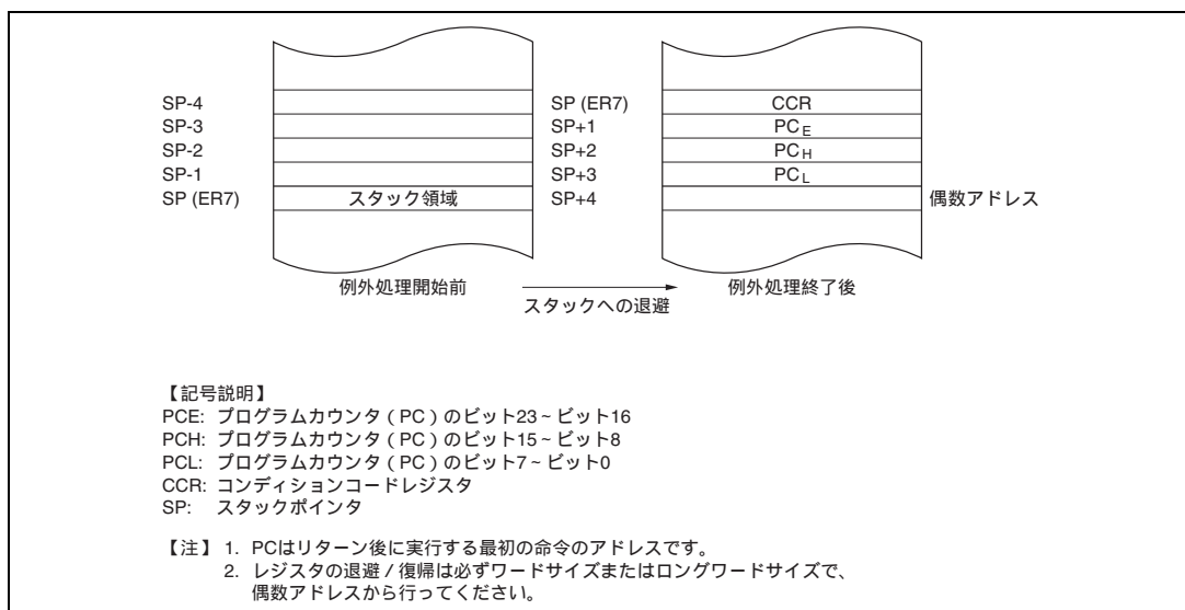
図 4.6 例外処理終了後のスタック状態
