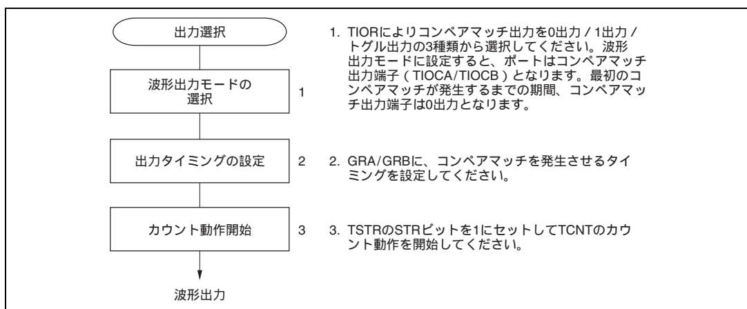
図 10.19 コンペアマッチによる波形出力動作例
