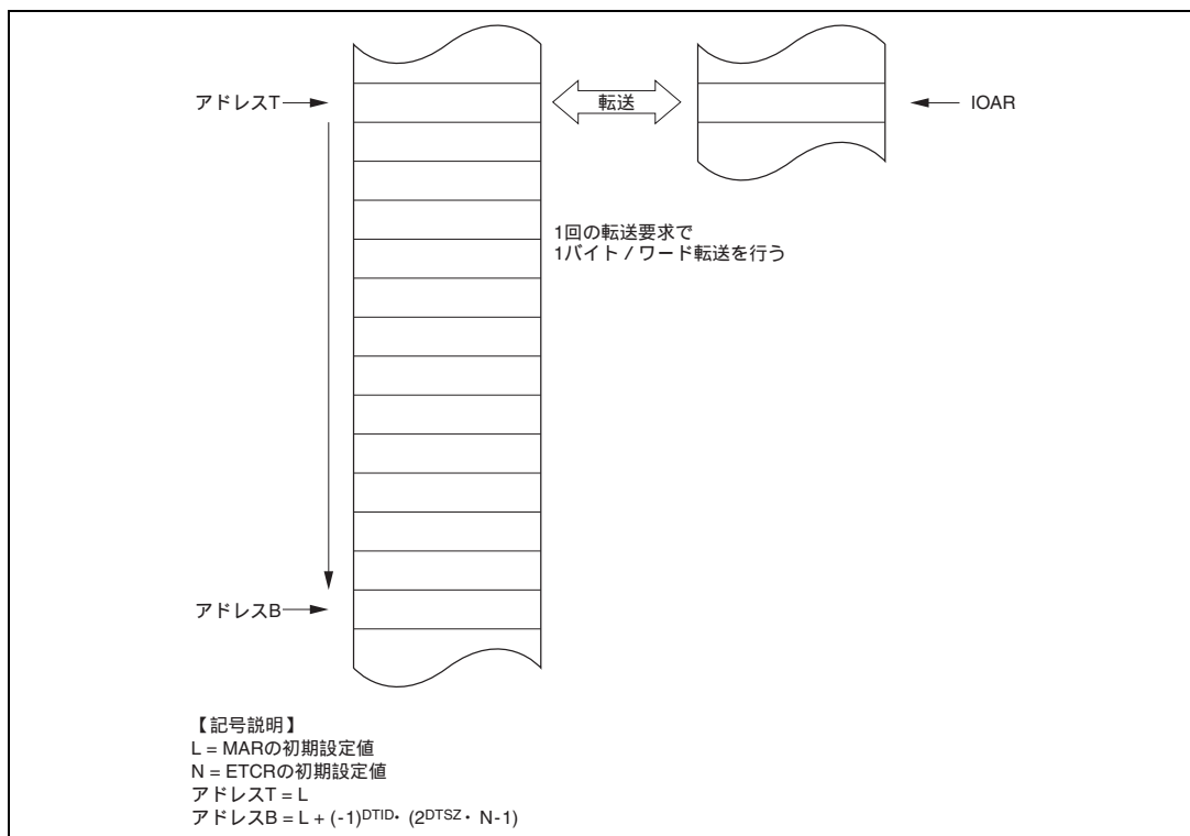
図 8.2 I/O モードの動作
