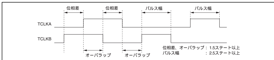
図 10.45 位相計数モード時の位相差、オーバーラップおよびパルス幅
