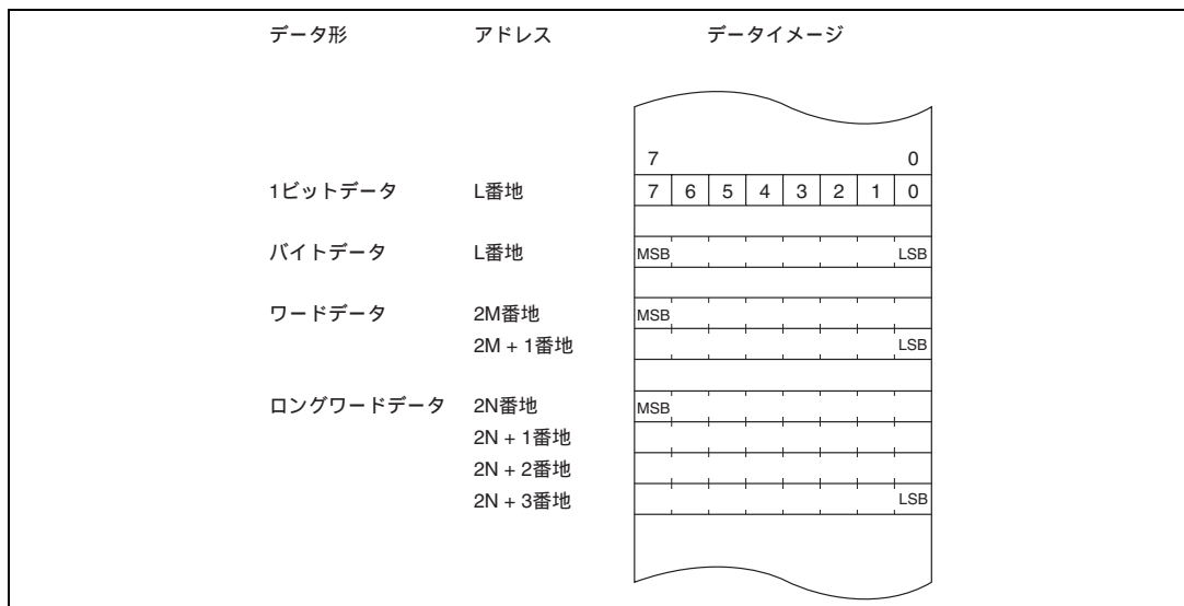
図 2.8 メモリ上でのデータ構成
