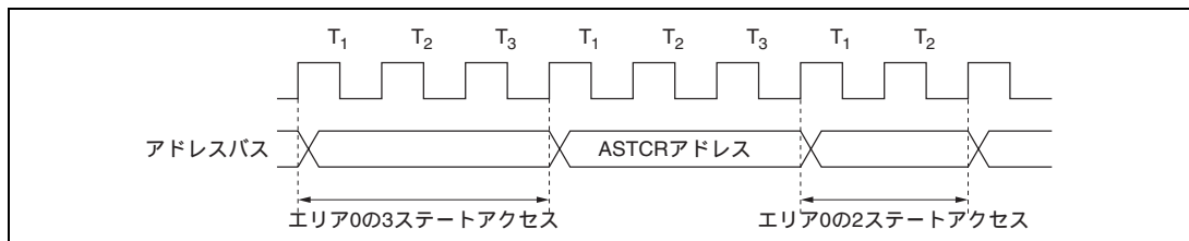
図 6.20 ASTCR ライトタイミング
