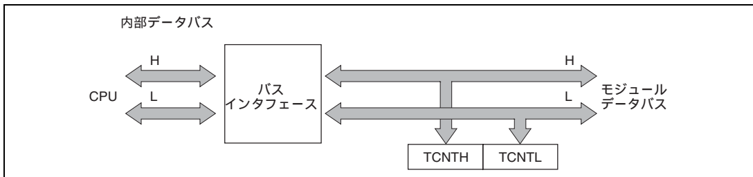
図 10.6 TCNT のアクセス動作 [ CPU TCNT (ワード) ]
