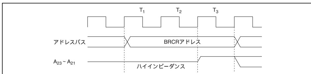
図 6.22 BRCR ライトタイミング
