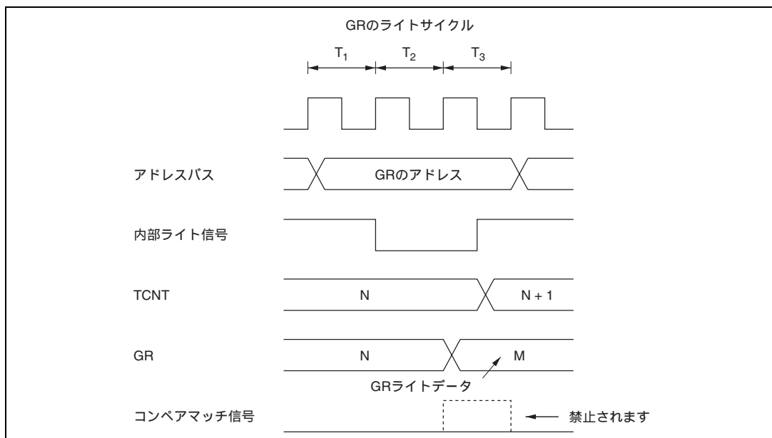
図 10.64 GRのライトとコンペアマッチの競合
