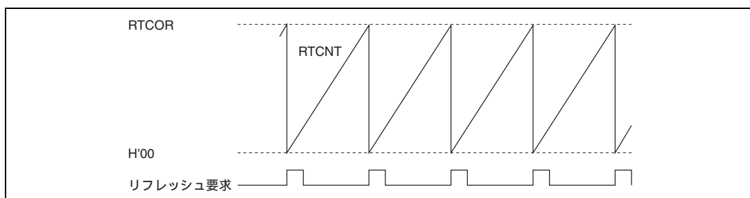
図 7.2 リフレッシュ要求の周期 (RCYCE = 1)
