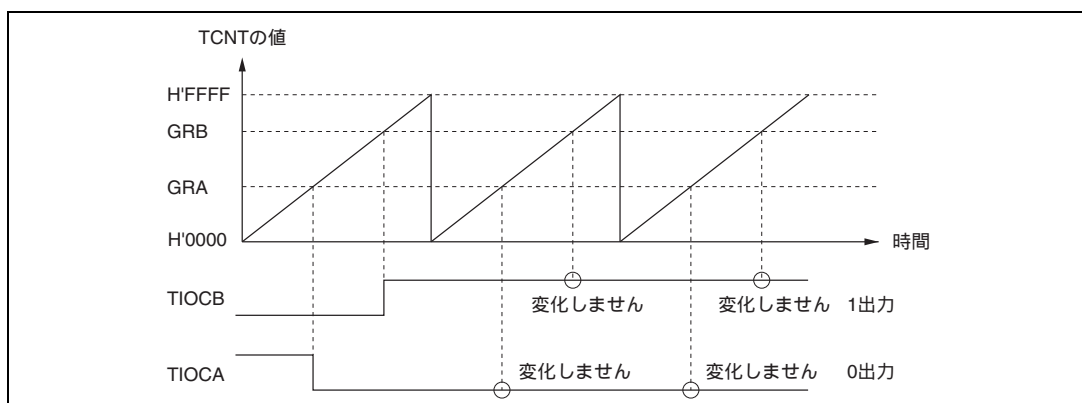
図 10.20 0 出力、1 出力の動作例
