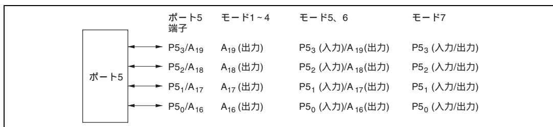
図 9.5 ポート5の端子構成
