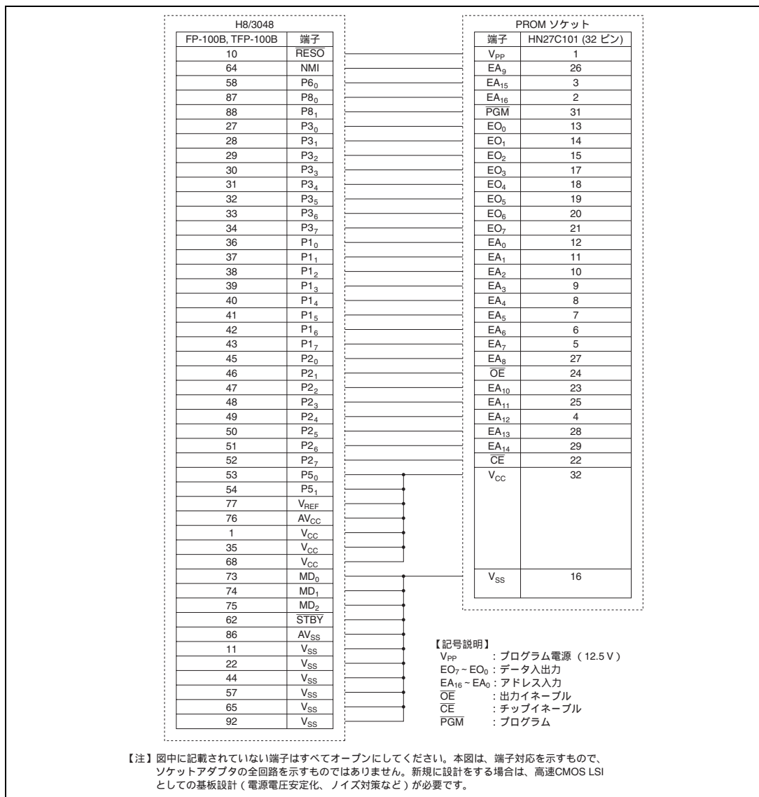
図 18.2 ソケットアダプタの端子対応図
