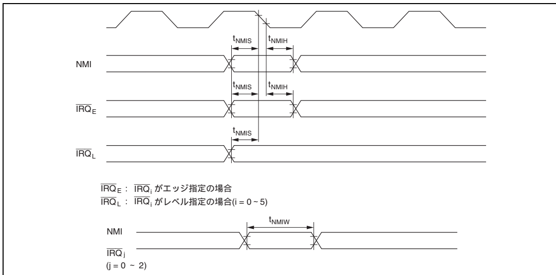
図 22.20 割り込み入力タイミング
