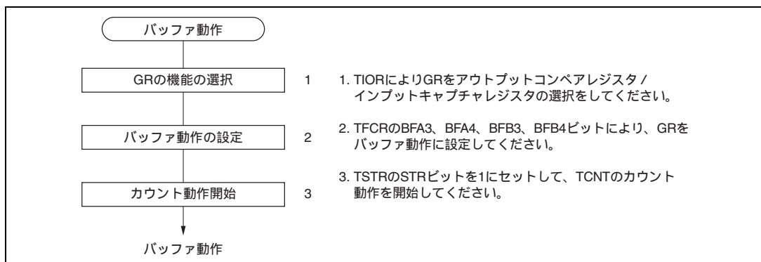
図 10.48 バッファ動作の設定手順例
