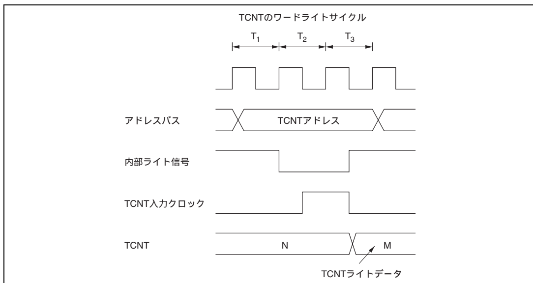
図 10.62 TCNTのワードライトとカウントアップの競合
