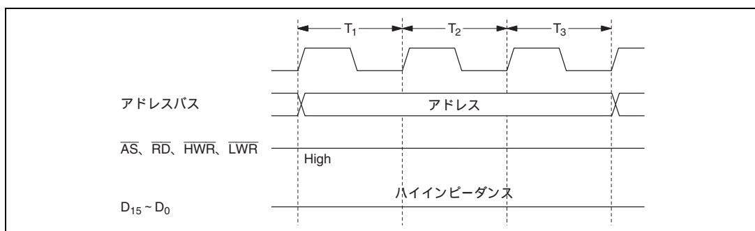
図 2.18 内蔵周辺モジュールアクセス時の端子状態
