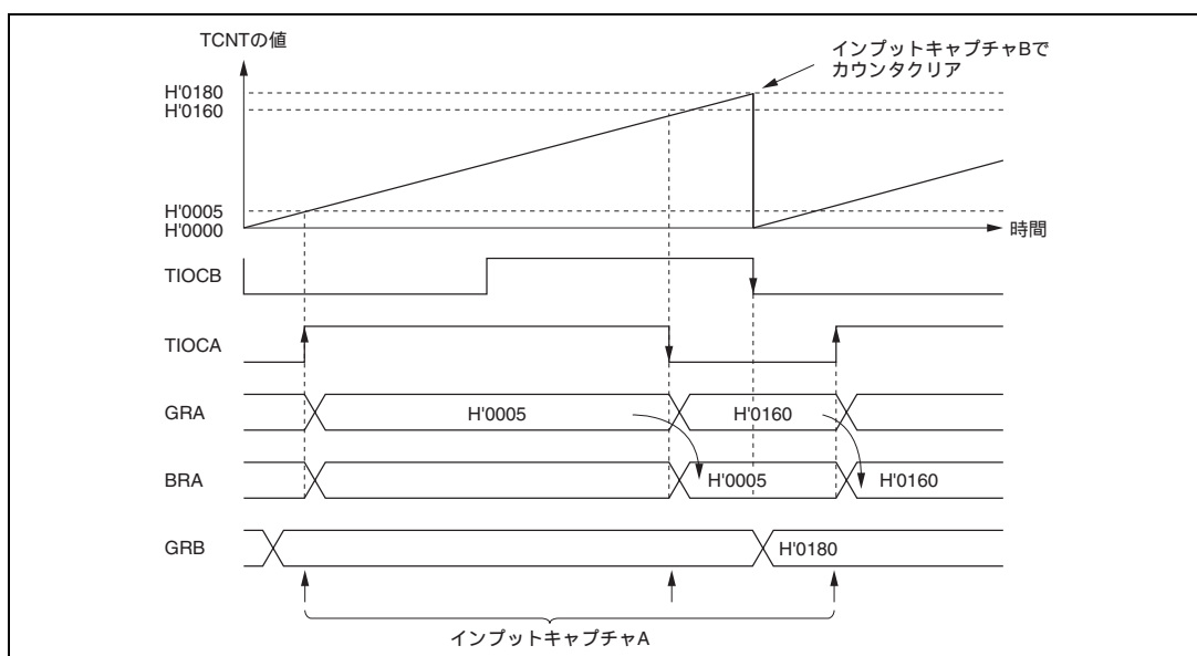
図 10.51 バッファ動作例 (2) (インプットキャプチャレジスタに対するバッファ動作)
