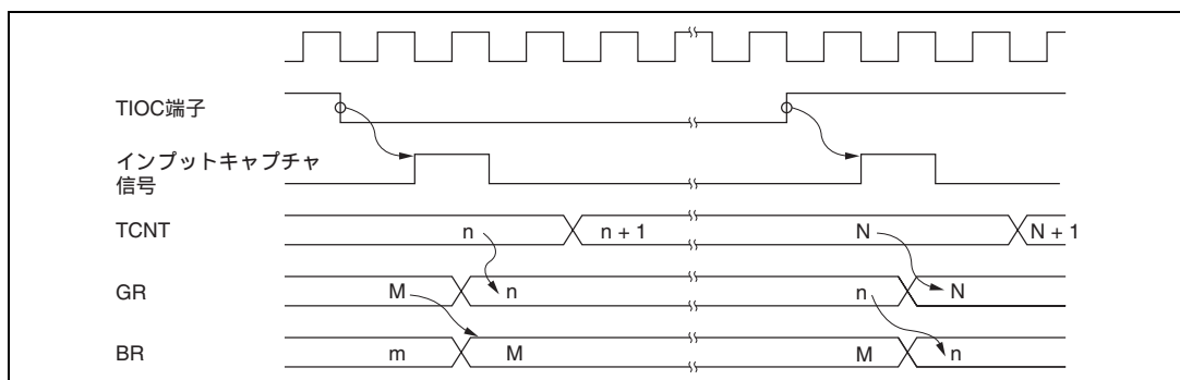
図 10.52 バッファ動作時のインプットキャプチャタイミング
