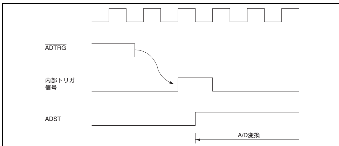
図 15.6 外部トリガ入力タイミング
