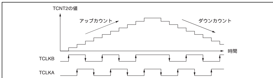
図 10.44 位相計数モードの動作例
