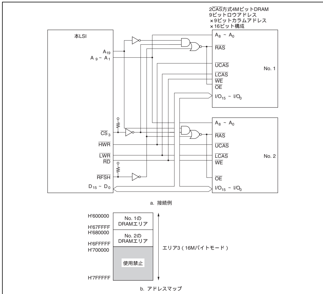
図 7.13 複数チップの2CAS方式4MビットDRAMの接続例とアドレスマップ
