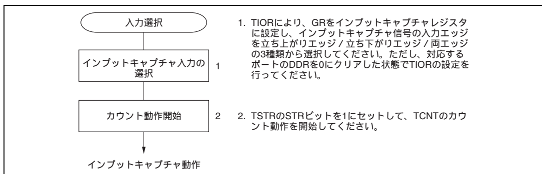
図 10.23 インพุットキャプチャ動作の設定手順例
