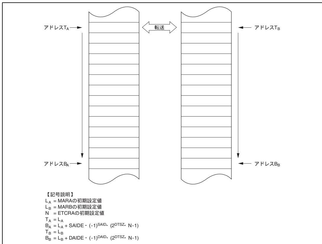
図 8.8 ノーマルモードの動作
