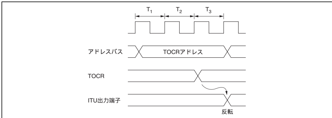
図 10.56 TOCR へのライトによる ITU 出力レベル反転タイミングの例
