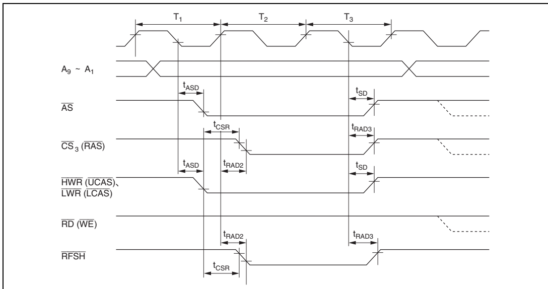
図 22.14 DRAM バスタイミング (リフレッシュサイクル時) / 3 ステートアクセス 2CAS 方式
