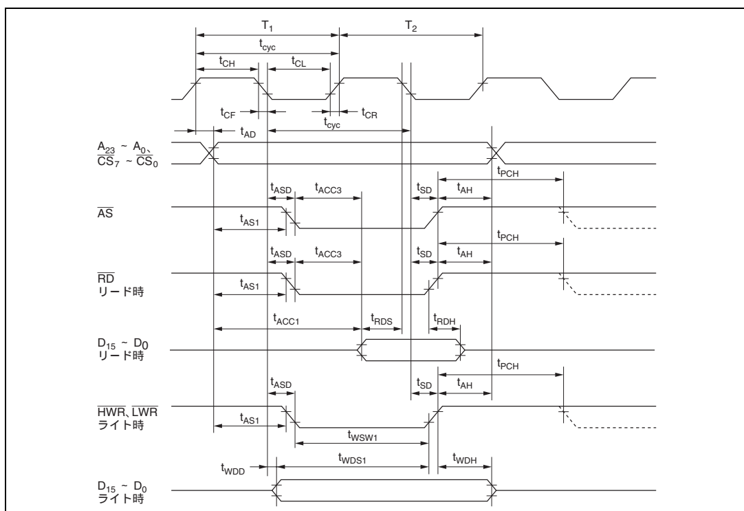
図 22.7 基本バスタイミング / 2 ステートアクセス
