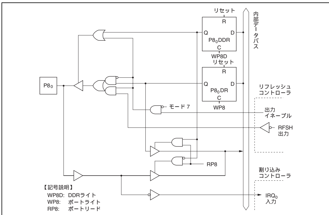
図C.8 (a) ポート 8 ブロック図 (P8 0 端子)
