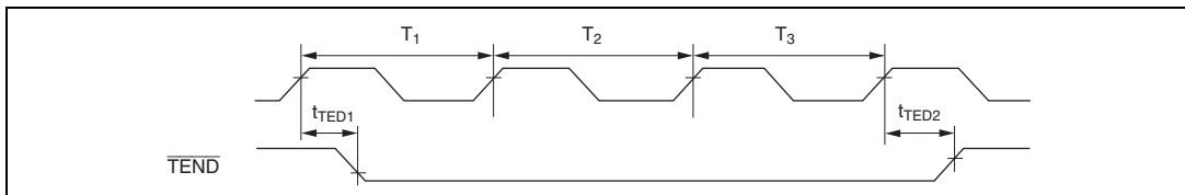
図 22.29 DMAC \overline{\text{TEND}} 出力タイミング / 3 ステートアクセス
