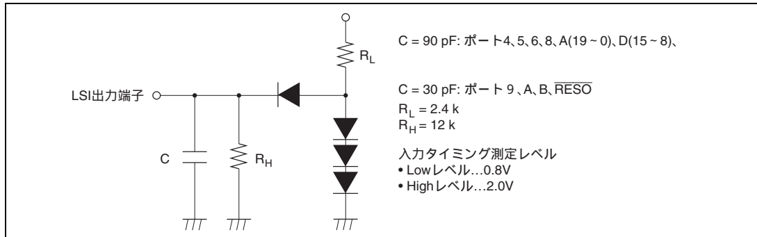
図 22.3 出力負荷回路
