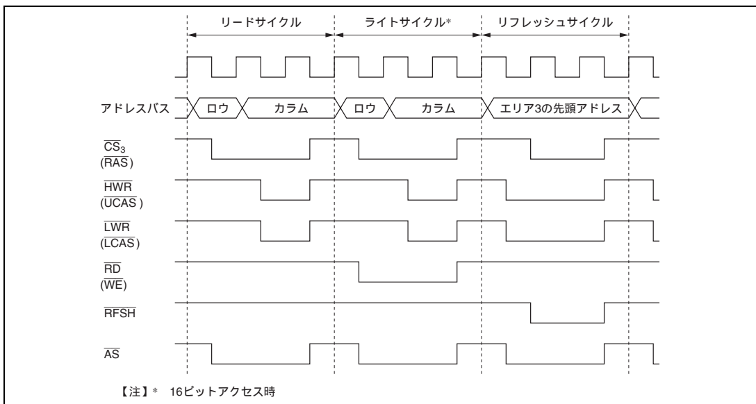
図 7.5 DRAM 制御信号出力タイミング (2) (2CAS 方式)
