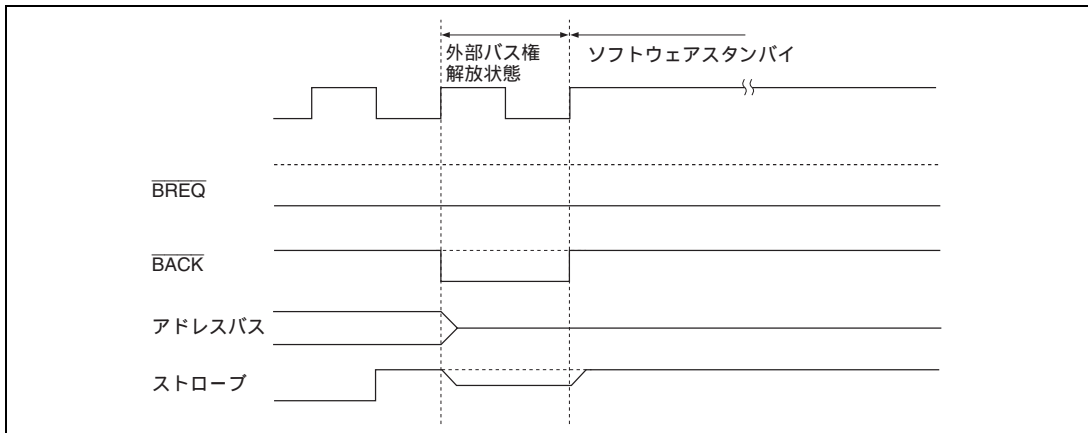
図 7.25 バス解放状態とソフトウェアスタンバイモードの競合
