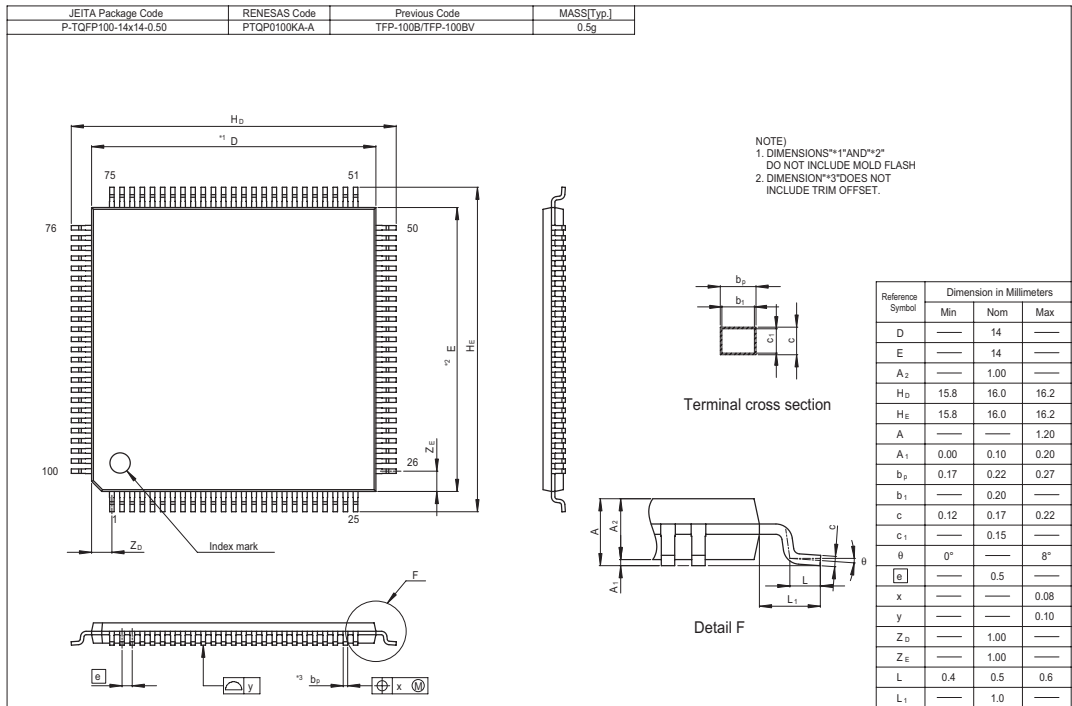
図 H.2 外形寸法図 (TFP-100B)
