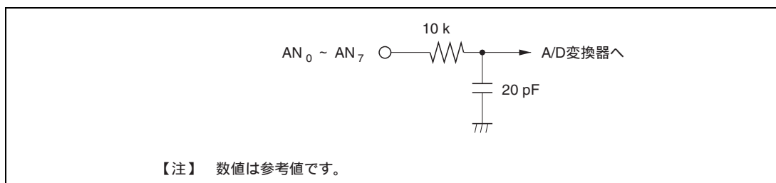
図 15.8 アナログ入力端子等価回路
