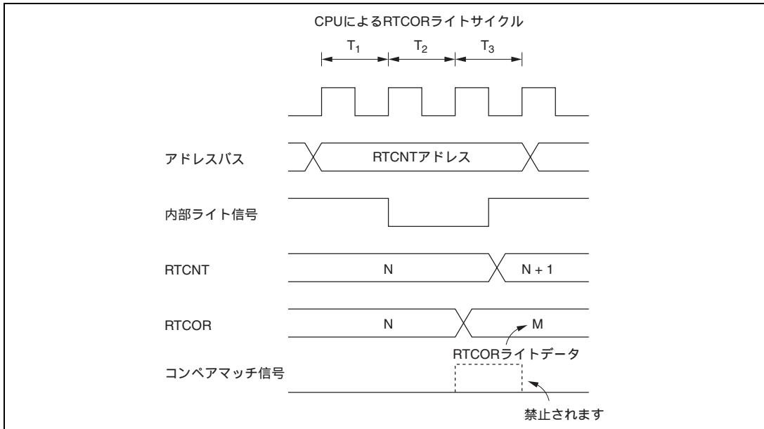
図 7.22 RTCOR のライトとコンペアマッチの競合
