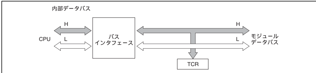
図 10.12 TCR のアクセス動作 [ CPU TCR ]
