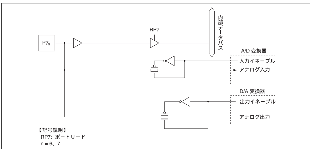
C.7 (b) ポート7ブロック図 (P7 6 ~ P7 7 端子)
