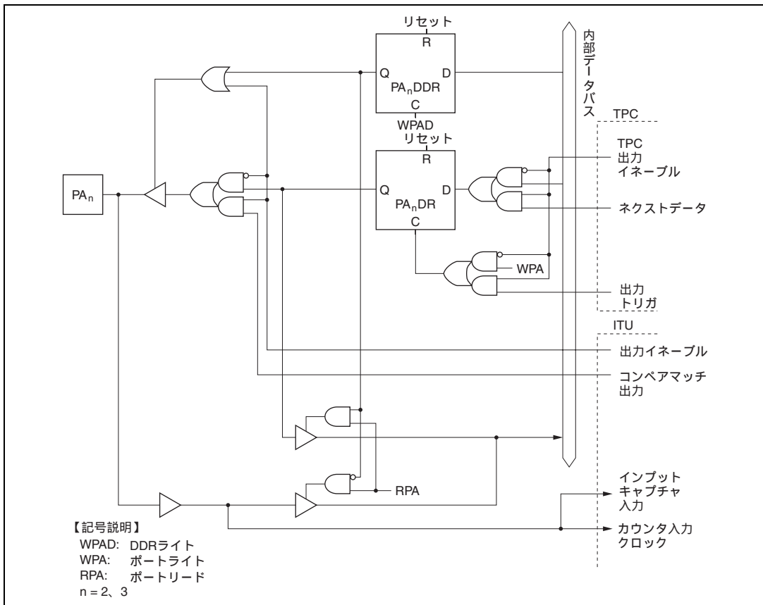
図C.10 (b) ポートAブロック図 (PA 2 , PA 3 端子)
