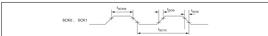
図 22.26 SCK 入力クロックタイミング
