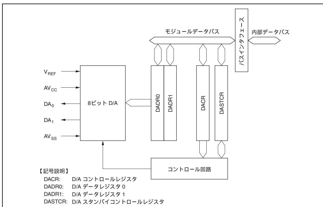
図 16.1 D/A 変換器のブロック図
