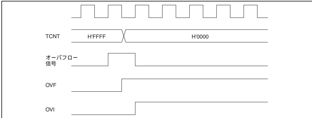
図 10.59 OVF フラグのセットタイミング
