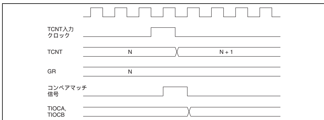
図 10.22 アウトプットコンペア出力タイミング
