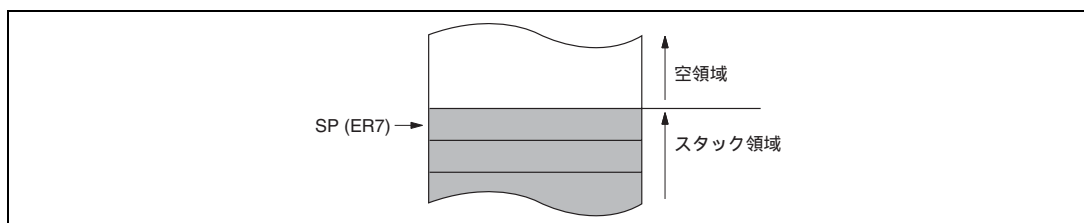
図 2.5 スタックの状態
