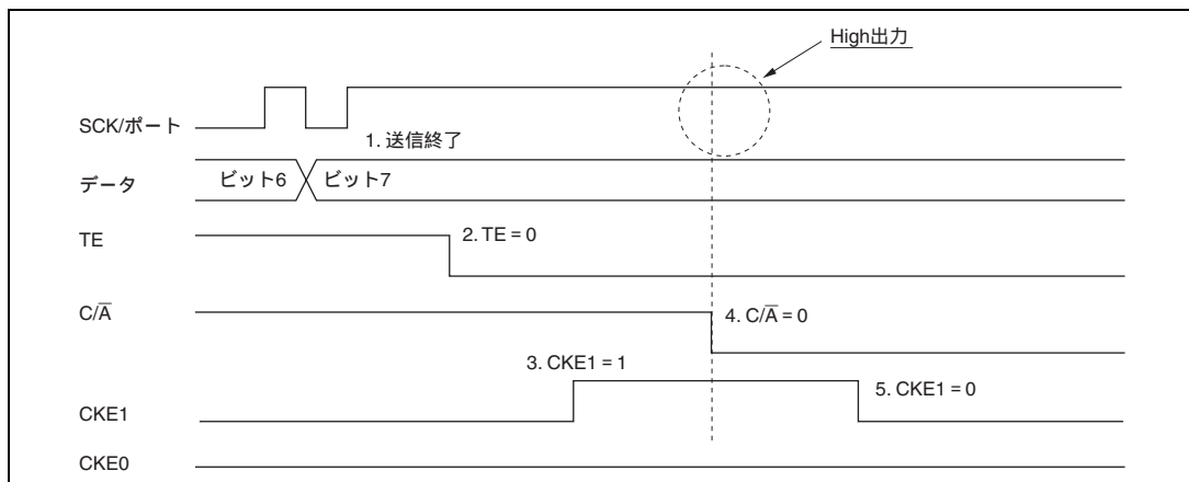
図 13.24 SCK 端子からポート端子へ切り替え時の動作 (Low 出力の回避例)
