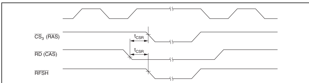
図 22.12 DRAM バスタイミング (セルフリフレッシュモード) 2WE 方式
