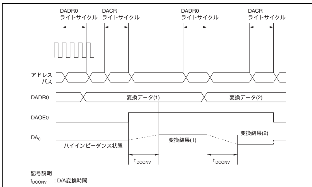
図 16.2 D/A 変換器の動作例
