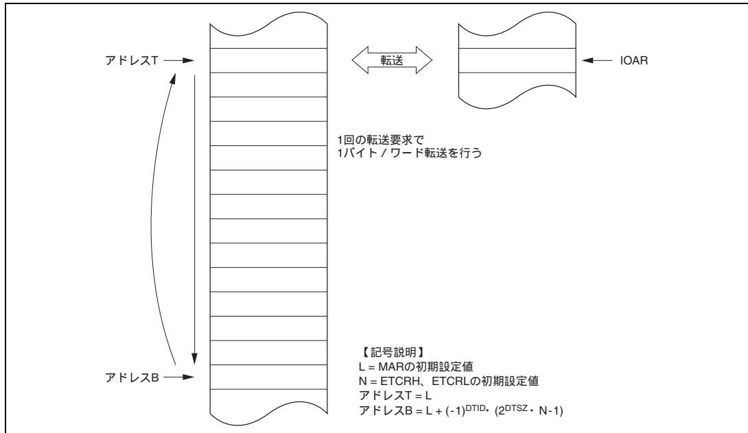
図 8.6 リピートモードの動作
