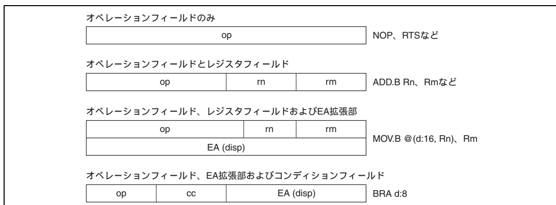
図 2.9 命令フォーマット
