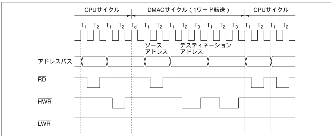
図 8.13 DMA 転送バスタイミング例
