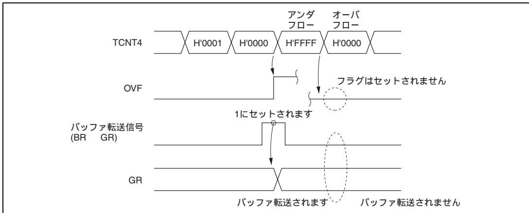
図 10.38 アンダシュート時のタイミング
