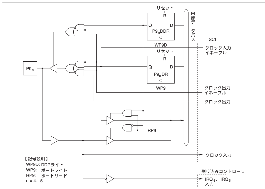
図C.9 (d) ポート9ブロック図 ( P9_4 、 P9_5 端子)
