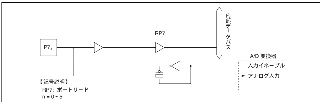
C.7 (a) ポート7ブロック図 (P7 0 ~ P7 5 端子)
