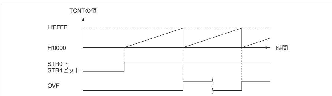
図 10.15 フリーランニングカウンタの動作
