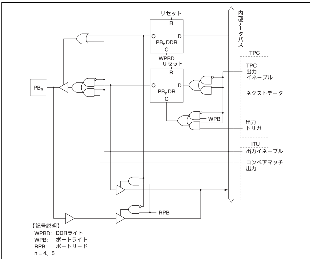
図C.11 (b) ポートBブロック図 (PB 4 , PB 5 端子)
