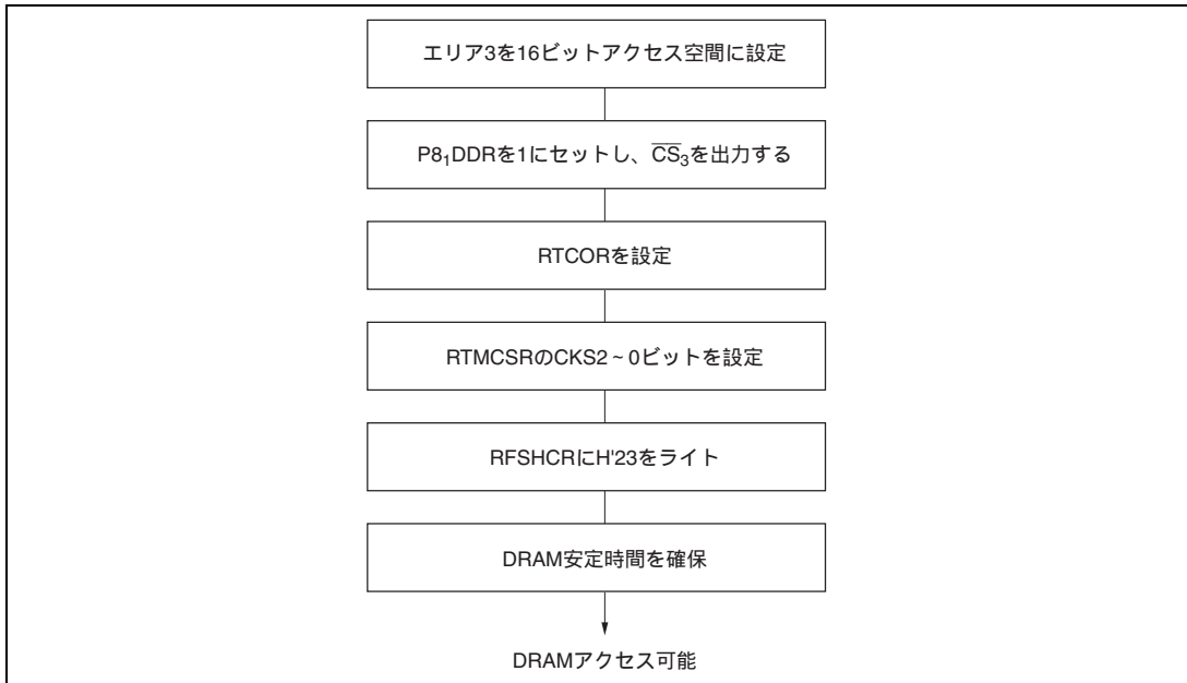
図 7.10 2WE 方式 4M ビット DRAM (10 ビットロウアドレス×8 ビットカラムアドレスの場合) の設定順序 (16M バイトモード)
