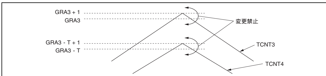
図 10.40 バッファ動作による GR の設定変更時の注意 ( 1 )
