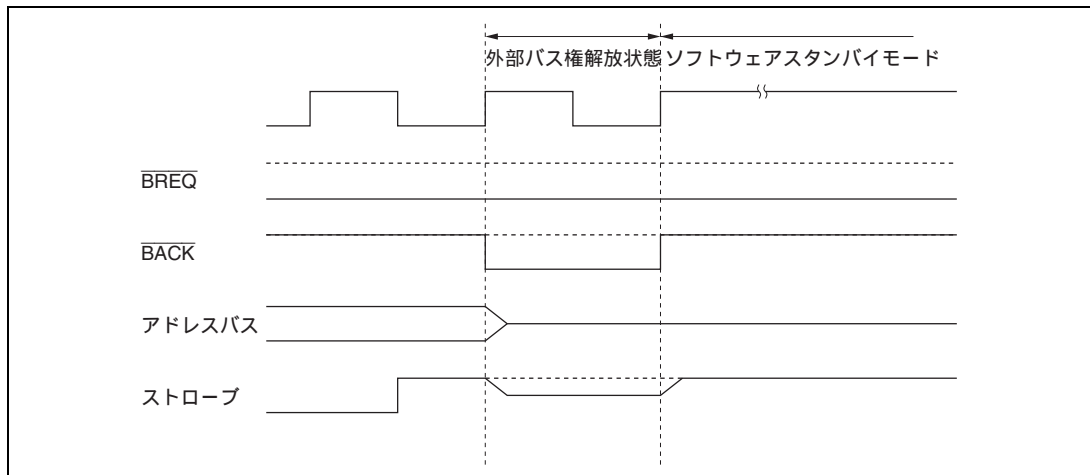
図 6.23 バス解放状態とソフトウェアスタンバイモードの競合
