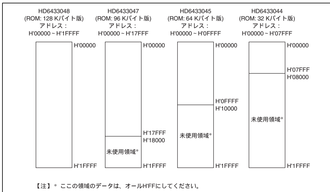
図 18.7 ROM アドレスとデータ
