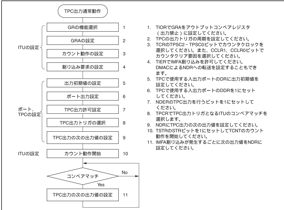
図 11.4 TPC 出力通常動作の設定手順例
