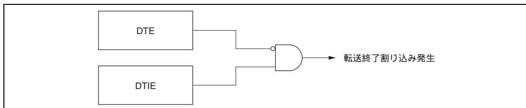
図 8.25 転送終了割り込みブロック図
