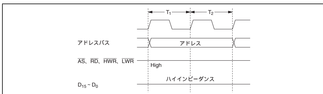
図 2.16 内蔵メモリアクセス時の端子状態
