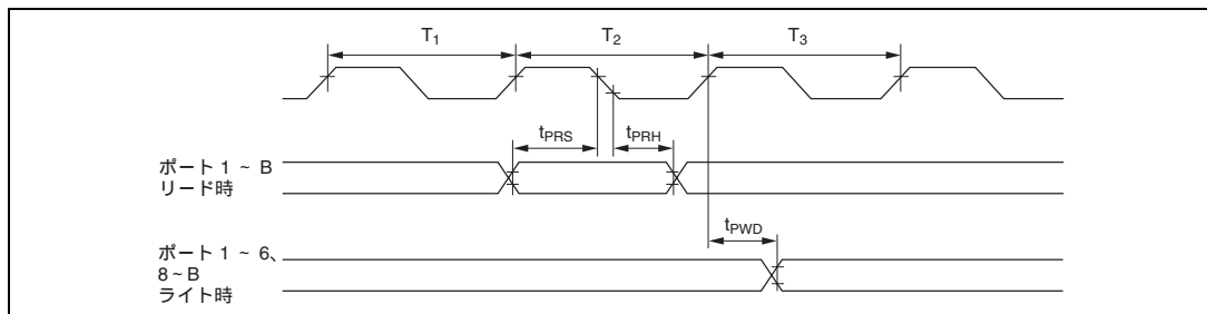
図 22.23 TPC、I/Oポート入出力タイミング
