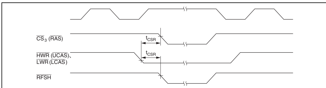
図 22.15 DRAM バスタイミング (セルフリフレッシュモード) 2CAS 方式
