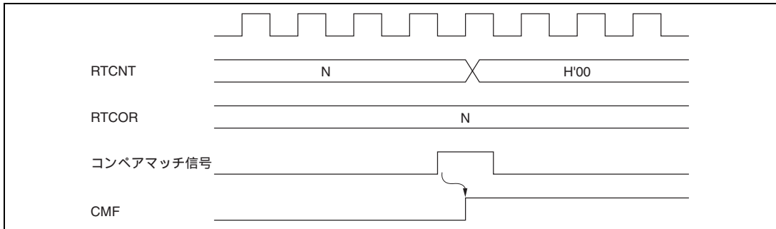
図 7.19 CMF フラグセットタイミング
