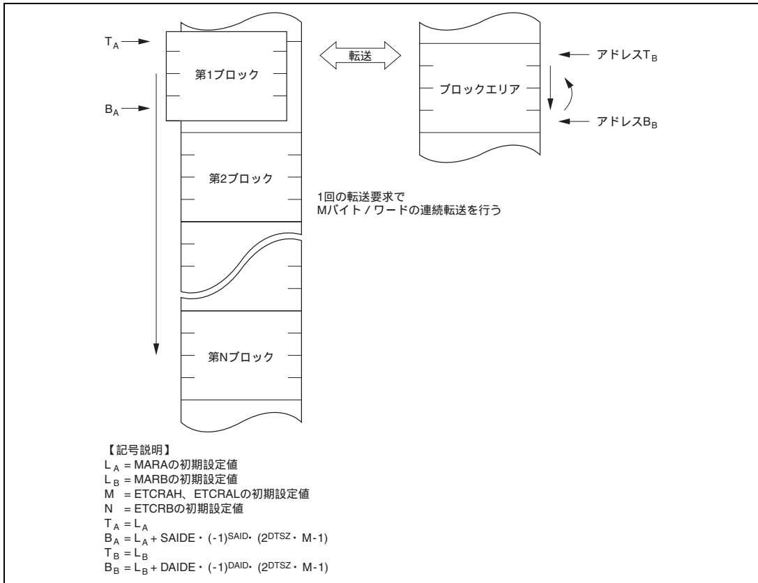
図 8.10 ブロック転送モードの動作
