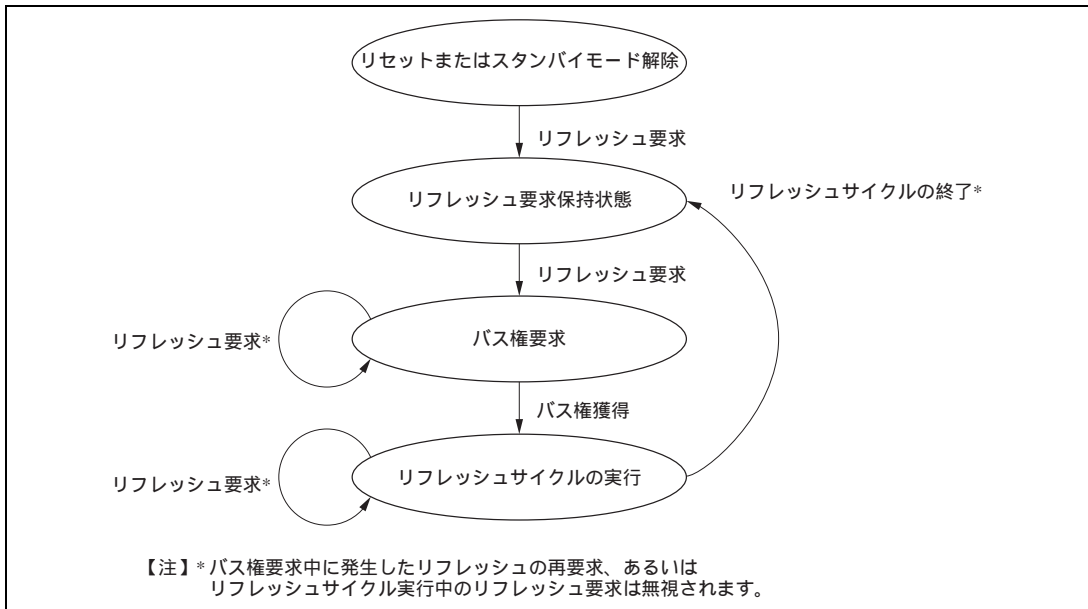
図 7.3 リフレッシュサイクル実行の状態遷移図
