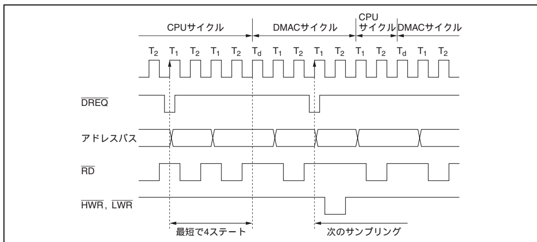
図 8.16 ノーマルモード時の \overline{\text{DREQ}} 端子の立ち下がりエッジによる DMAC 起動タイミング
