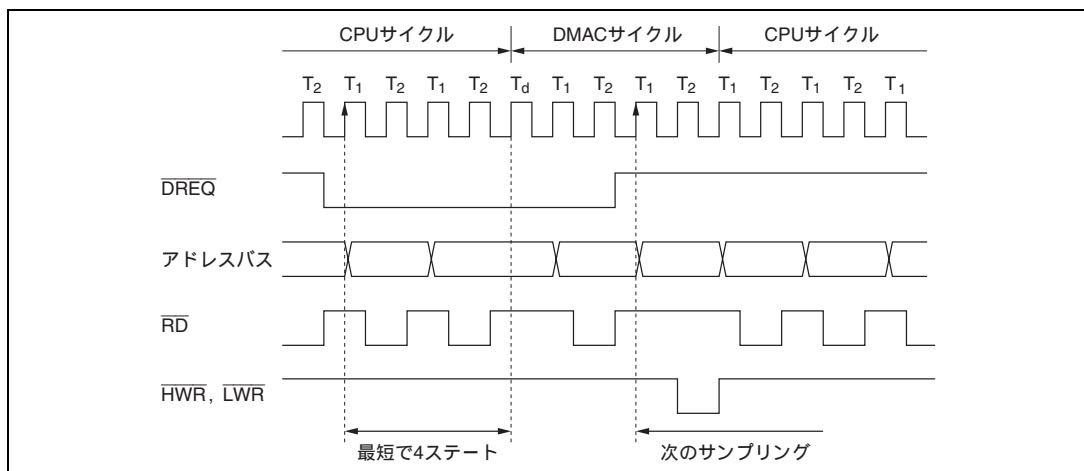
図 8.17 ノーマルモード時の \overline{\text{DREQ}} 端子の Low レベルによる DMAC 起動タイミング
