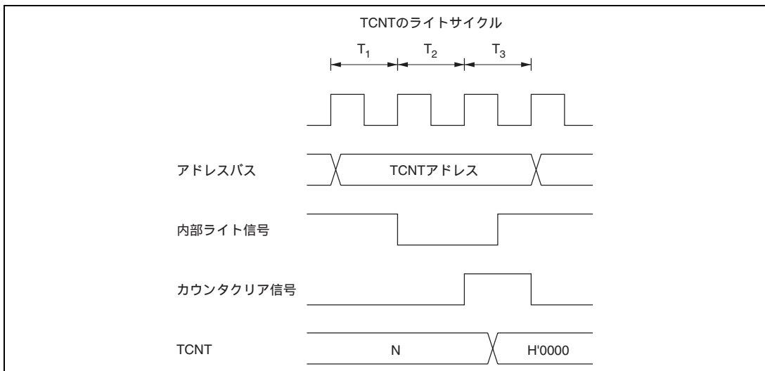
図 10.61 TCNT のライトとクリアの競合
