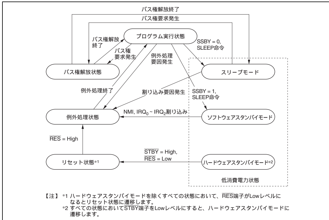
図 2.13 状態遷移図
