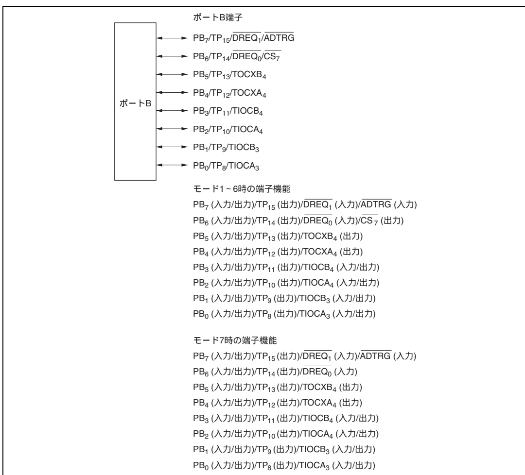
図 9.11 ポート B の端子構成
