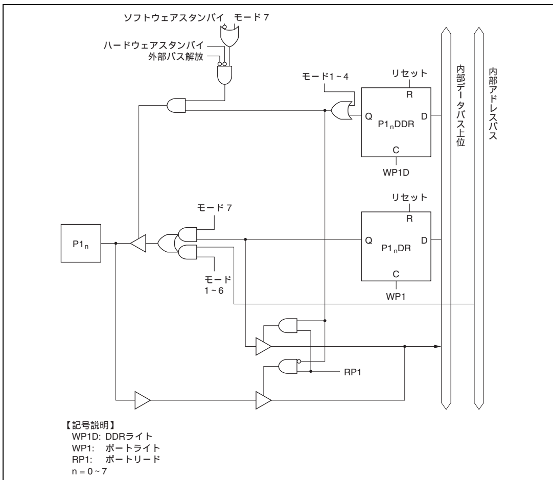
図 C.1 ポート1ブロック図
