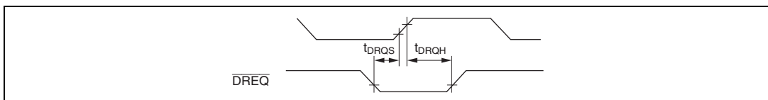
図 22.30 DMAC \overline{\text{DREQ}} 入力タイミング
