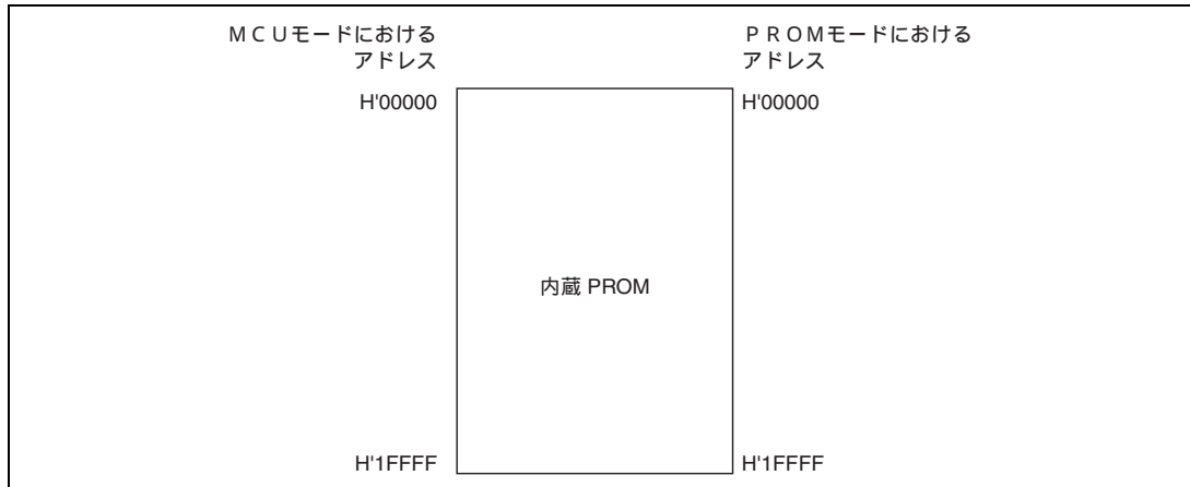
図 18.3 H8/3048ZTAT の PROM モード時のメモリマップ
