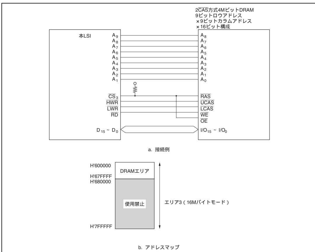
図 7.11 2 \overline{\text{CAS}} 方式 4M ビット DRAM の接続例とアドレスマップ
