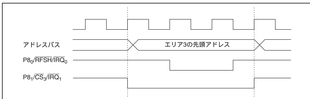
図 7.23 DRAM/PSRAM 接続の切り離し時の動作
