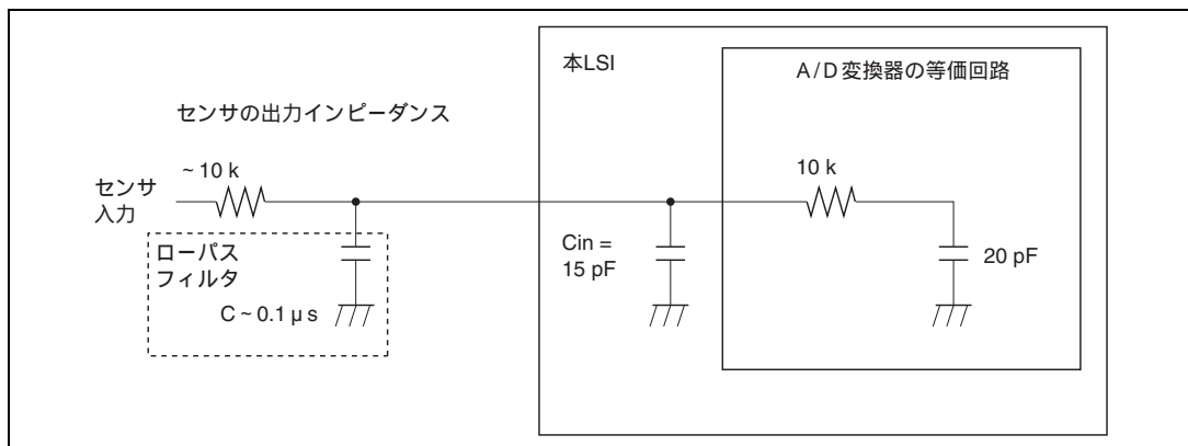
図 15.11 アナログ入力回路の例
