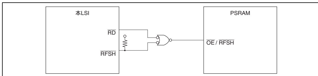
図 7.17 OE / RFSH 信号の例
