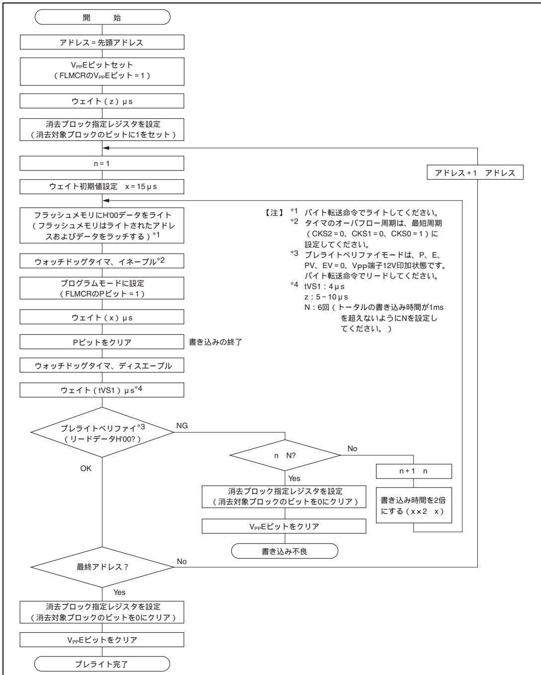
図 19.11 プレライトフローチャート
