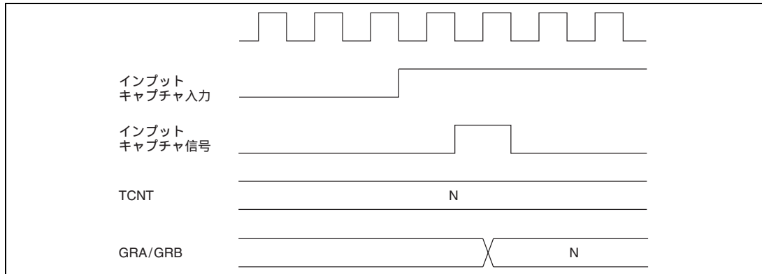
図 10.25 インพุットキャプチャ入力信号タイミング
