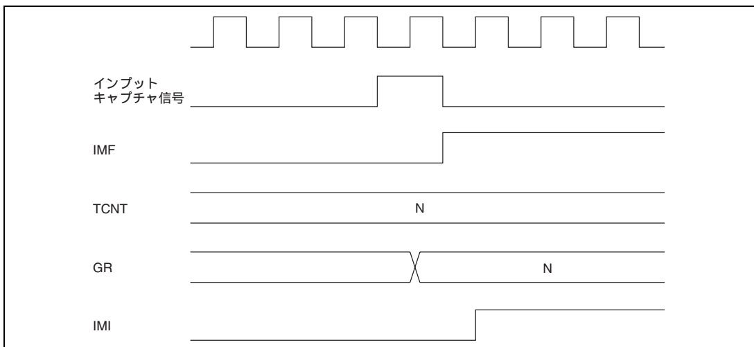
図 10.58 インพุットキャプチャ時の IMFA、IMFB フラグのセットタイミング
