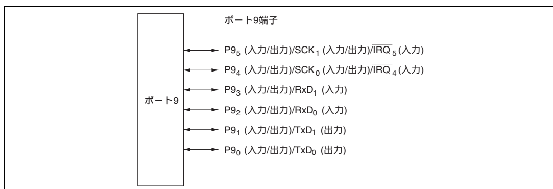
図 9.9 ポート 9 の端子構成
