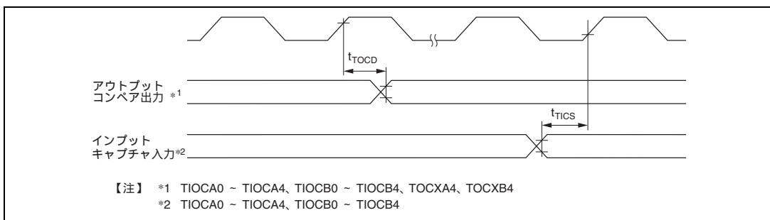
図 22.24 ITU 入出力タイミング
