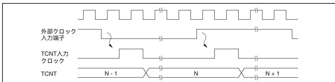
図 10.18 外部クロック動作時のカウントタイミング (両エッジ検出の場合)
