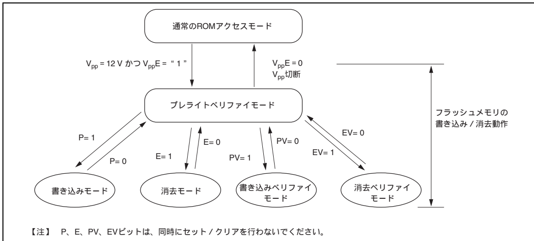
図 19.8 フラッシュメモリ書き込み / 消去動作モードの状態遷移図
