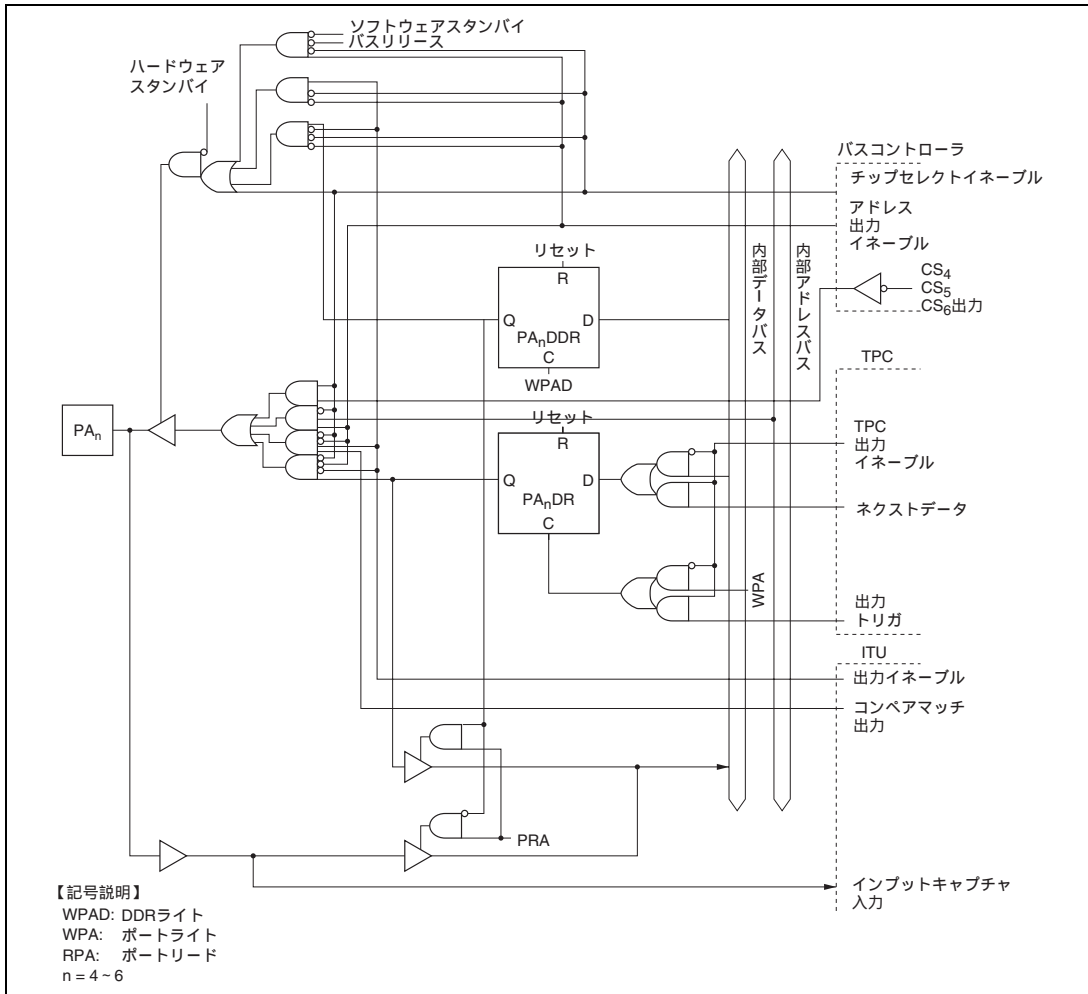
図C.10 (c) ポートAブロック図 (PA 4 ~ PA 6 端子)
