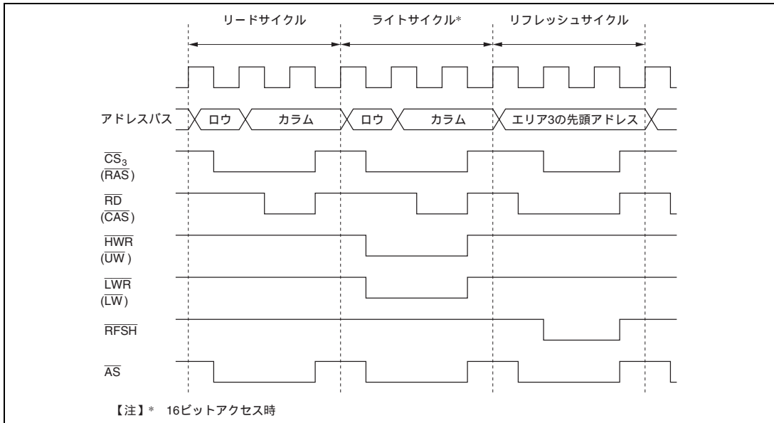
図 7.5 DRAM 制御信号出力タイミング (1) (2WE 方式)
