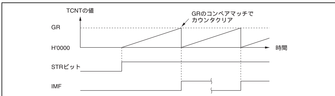
図 10.16 周期カウンタの動作
