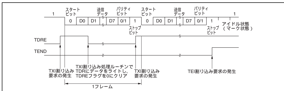
図 13.6 調歩同期式モードでの送信時の動作例 (8ビットデータ/パリティあり/1ストップビットの例)
