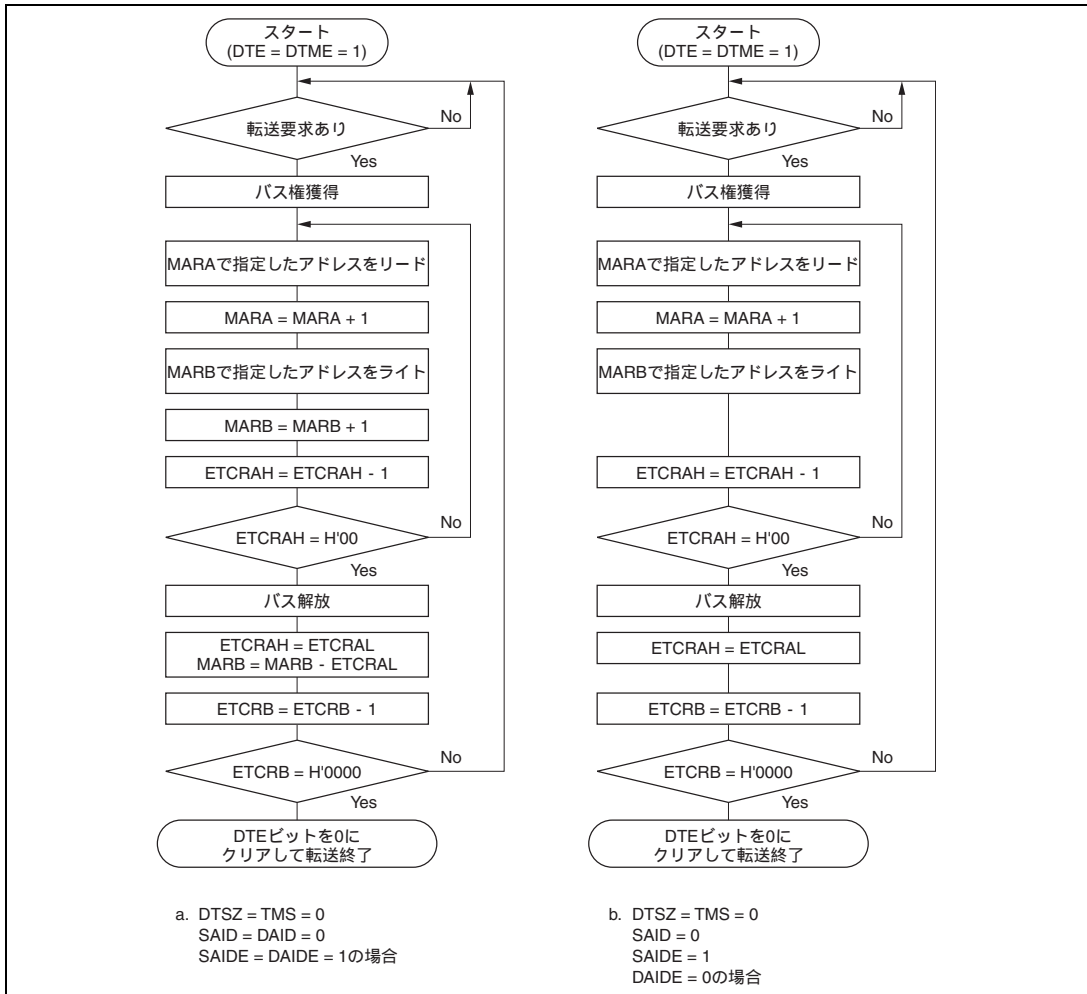
図 8.11 ブロック転送モードの動作フロー例
