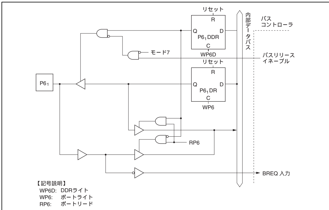
図C.6 (b) ポート6ブロック図 (P6 1 端子)
