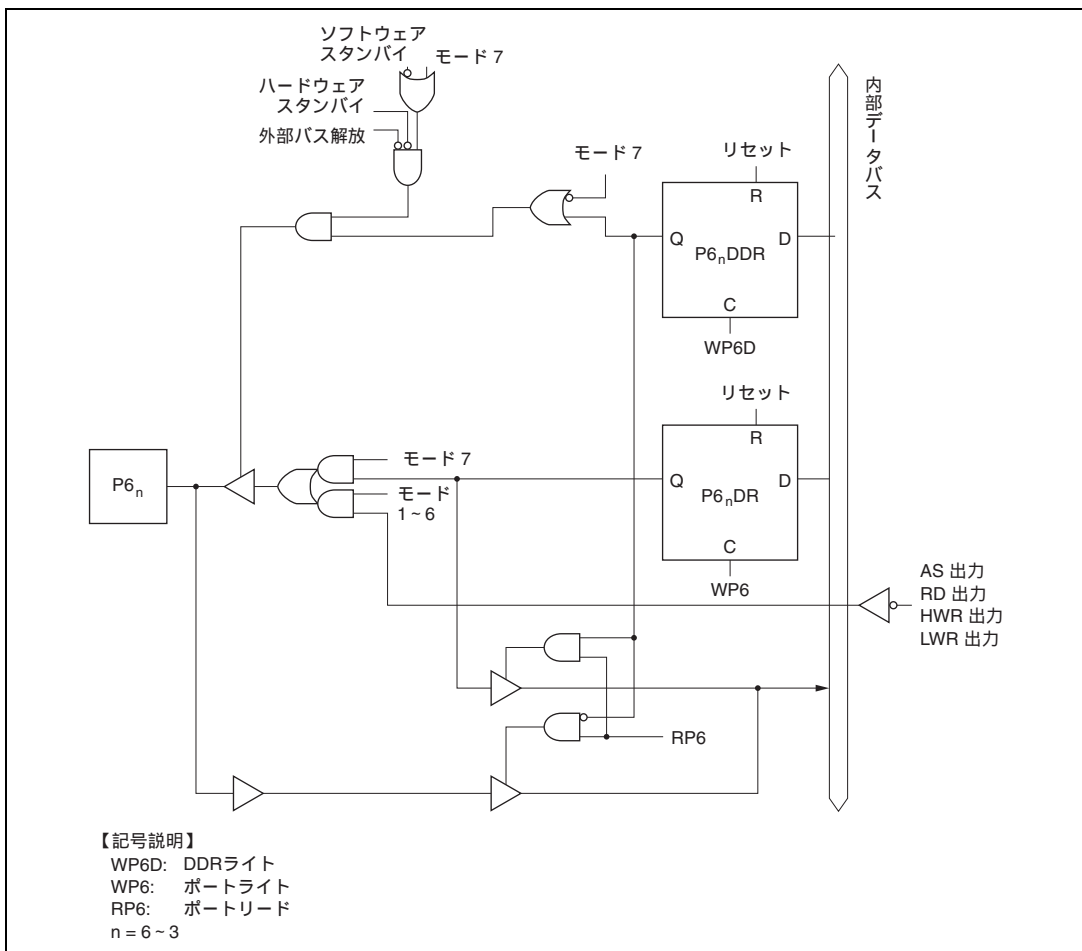
図C.6 (d) ポート 6 ブロック図 (P6 6 ~ P6 3 端子)
