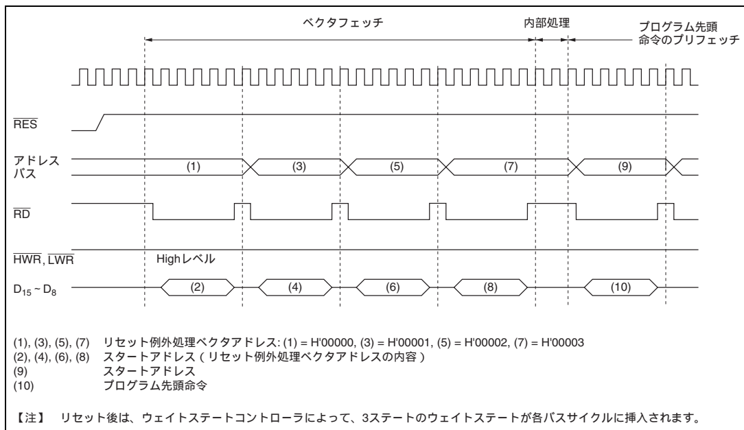
図 4.2 リセットシーケンス (モード 1、3)
