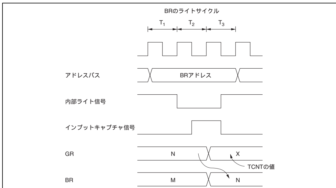
図 10.69 BR のライトとインプットキャプチャの競合
