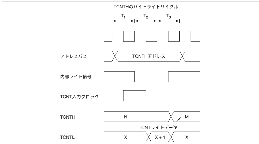
図 10.63 TCNT のバイトライトとカウントアップの競合
