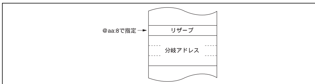
図 2.10 メモリ間接による分岐アドレスの指定
