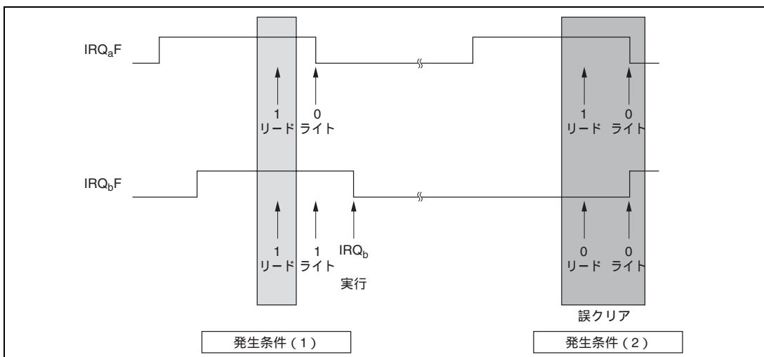
図 5.9 割り込み例外処理が実行されない場合のIRQ n Fフラグ
