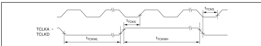
図 22.25 ITU 外部クロック入力タイミング
