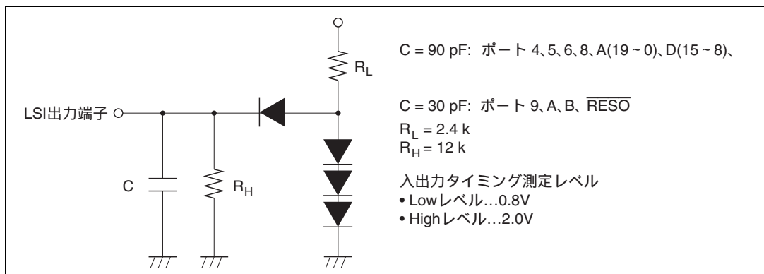
図 22.6 出力負荷回路
