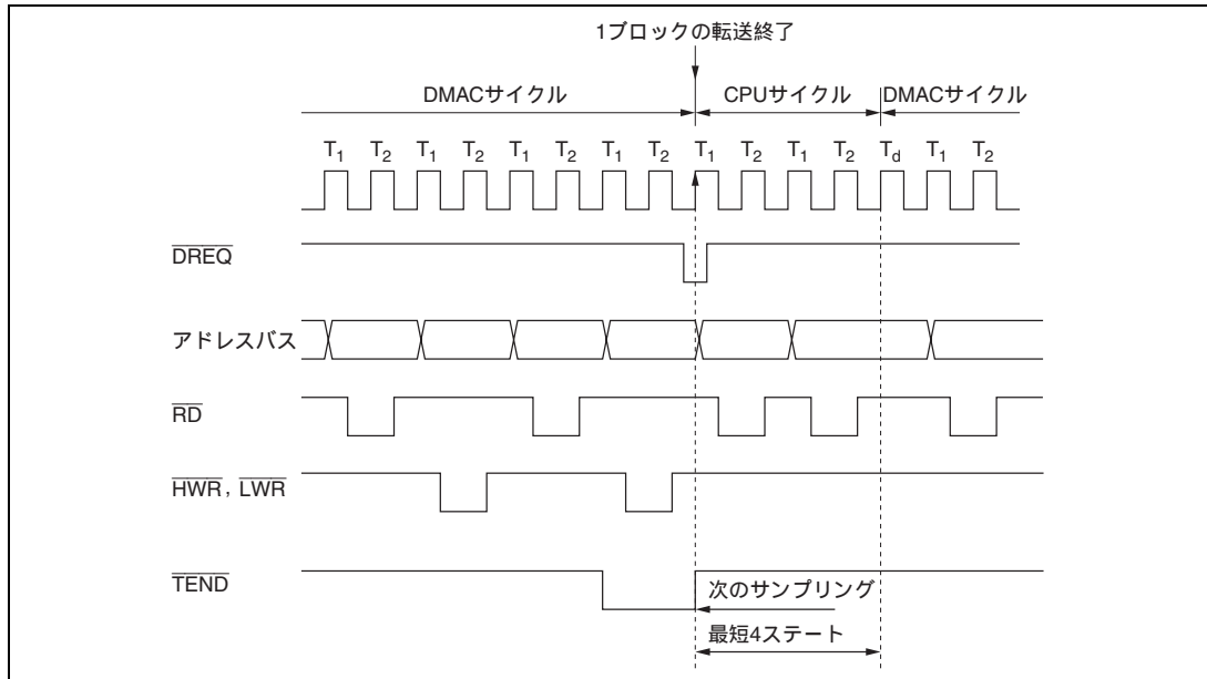
図 8.18 ブロック転送モード時の \overline{\text{DREQ}} 端子の立ち下がりエッジによる DMAC 起動タイミング
