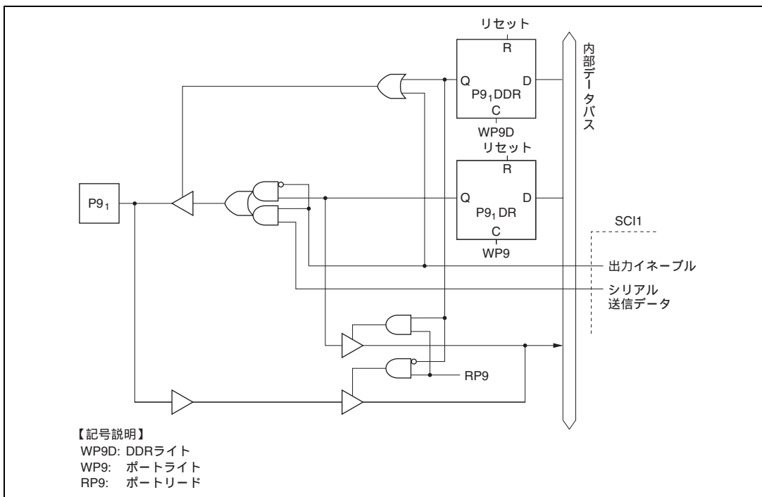
図C.9 (b) ポート9ブロック図 (P9 1 端子)
