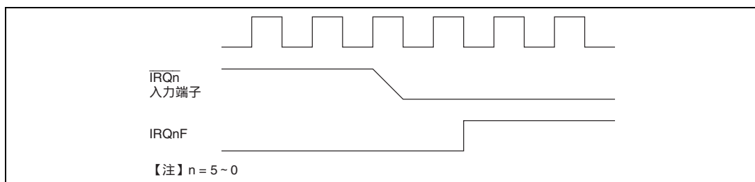
図 5.3 IRQnF セットタイミング
