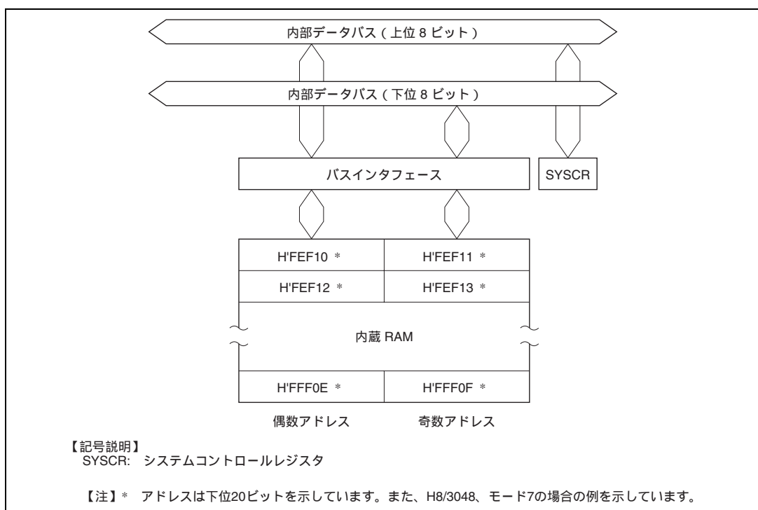
図 17.1 RAM のブロック図
