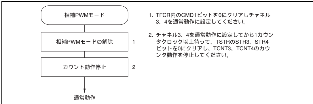
図 10.34 相補 PWM モードの解除手順
