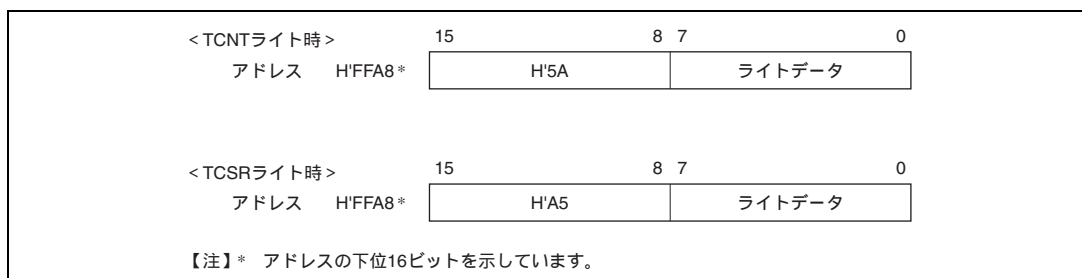
図 12.2 TCNT、TCSR へのライトデータ
