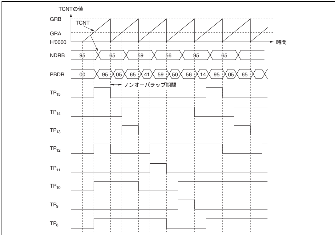
図 11.7 TPC 出力ノンオーバーラップ動作例 (4相の相補ノンオーバーラップ出力例)
