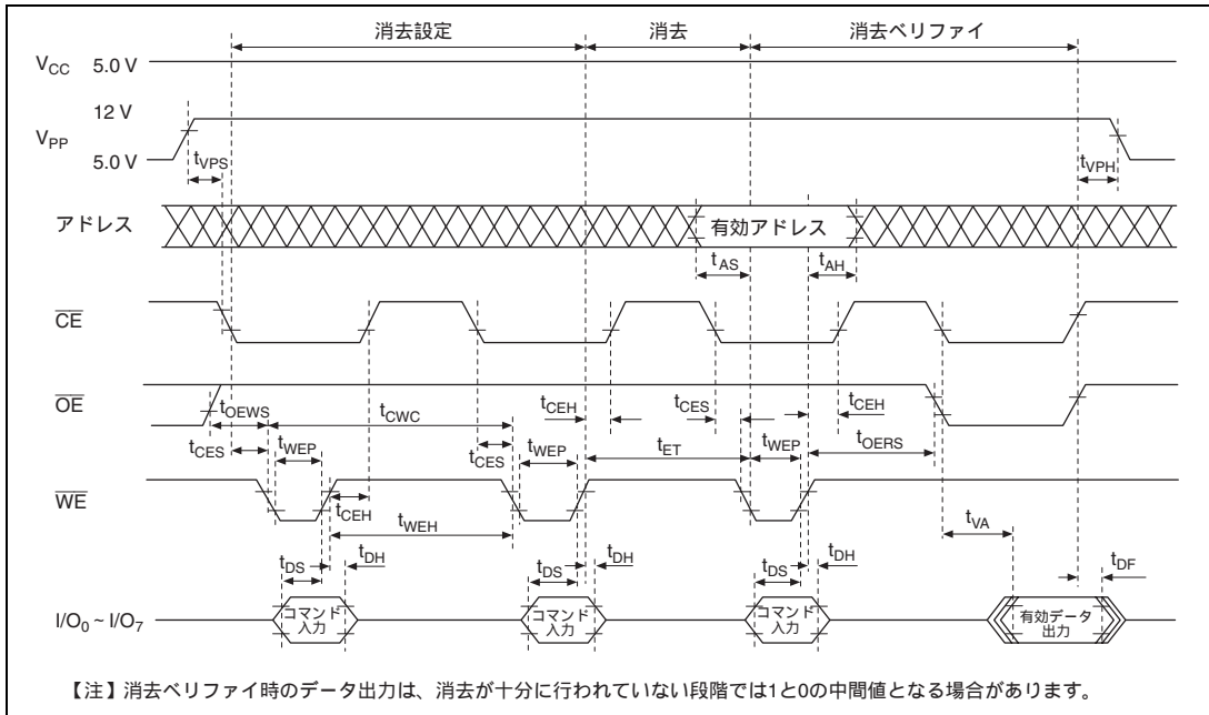
図 19.21 消去タイミング
