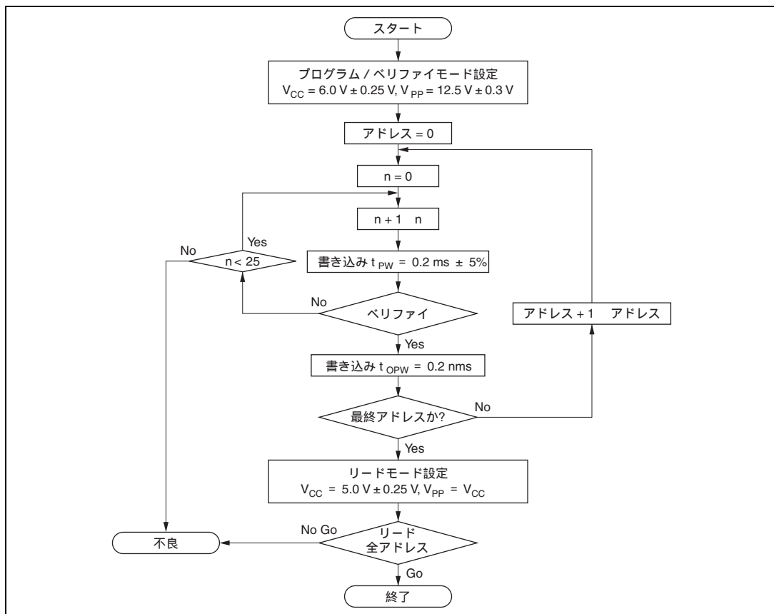
図 18.4 高速プログラミングフローチャート
