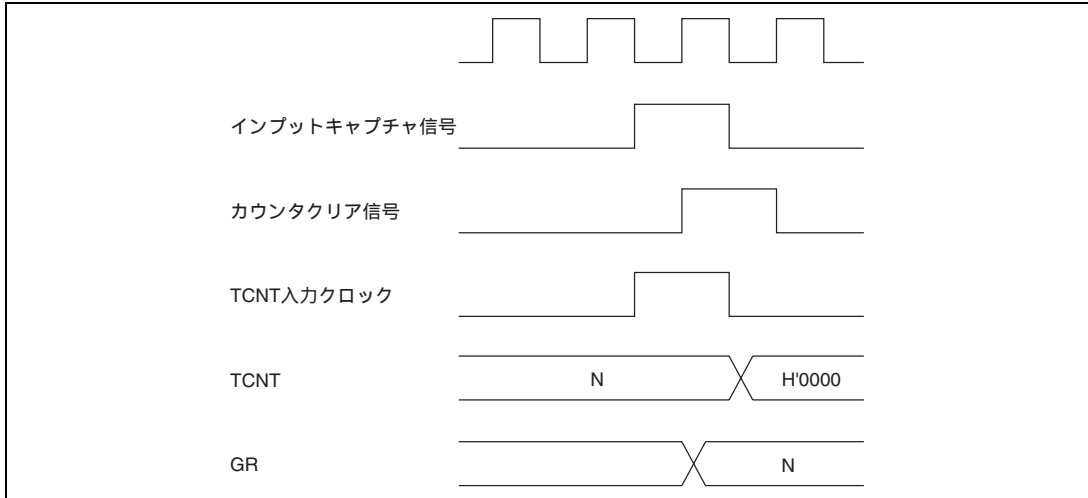
図 10.67 インพุットキャプチャによるカウンタクリアとカウントアップの競合
