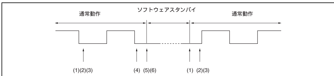
図 14.9 クロック停止・再起動手順
