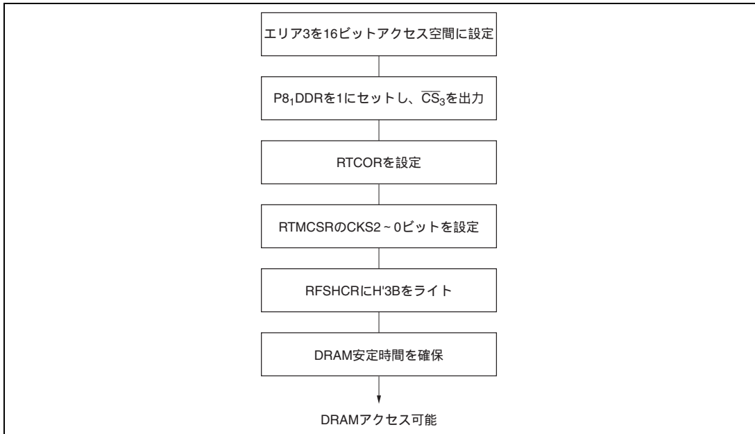
図 7.12 2CAS 方式 4M ビット DRAM (9 ビットロウアドレス×9 ビットカラムアドレスの場合) の設定順序 (16M バイトモード)
