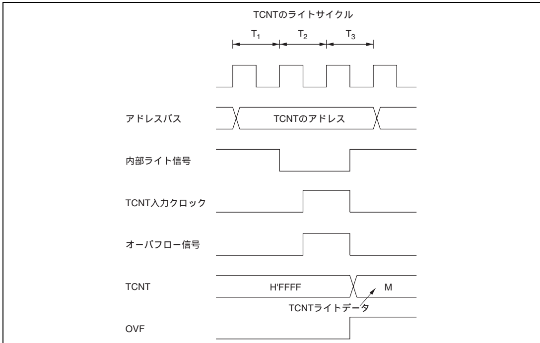
図 10.65 TCNT のライトとオーバーフローの競合
