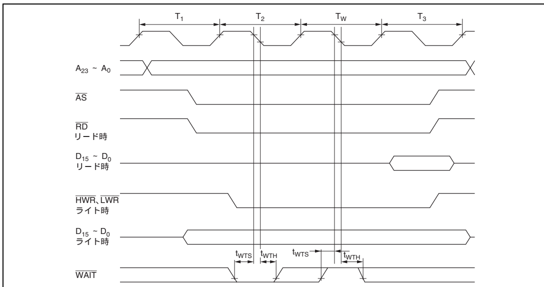
図 22.9 基本バスタイミング / 3 ステートアクセス 1 ウェイト
