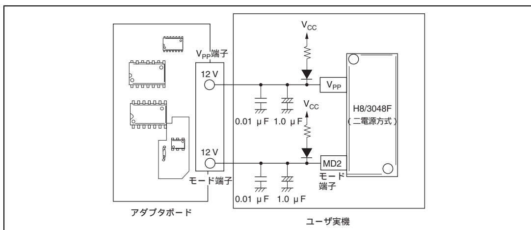
図 19.26 二電源方式のH8/3048F-ZTATの実装基板設計例 (アダプタボードとの接続) ( V_{pp} 端子とモード端子の設定が1の場合)
