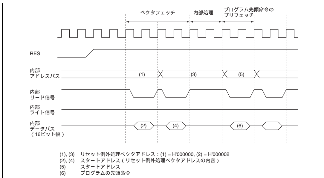
図 4.4 リセットシーケンス (モード 5、6、7)
