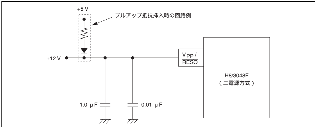
図 19.25 V_{pp} 電源回路設計例
