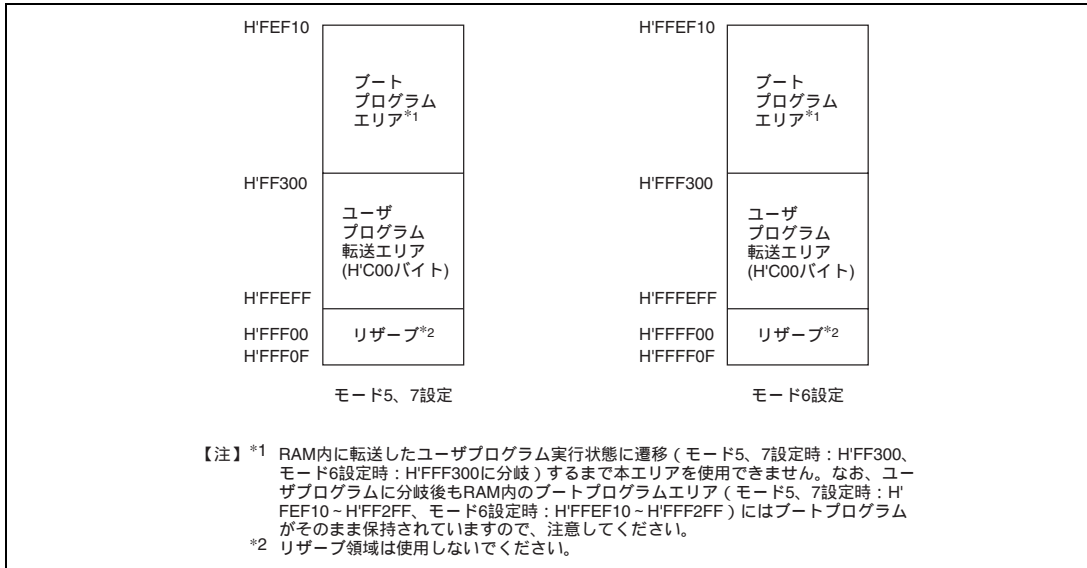
図 19.6 ブートモード時の RAM エリア
