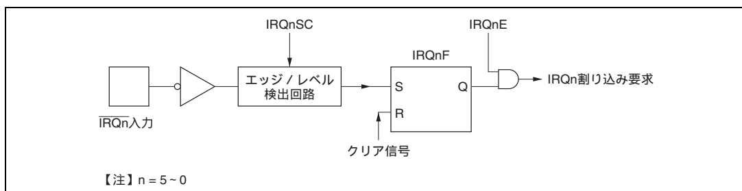
図 5.2 IRQ 0 ～IRQ 5 割り込みのブロック図
