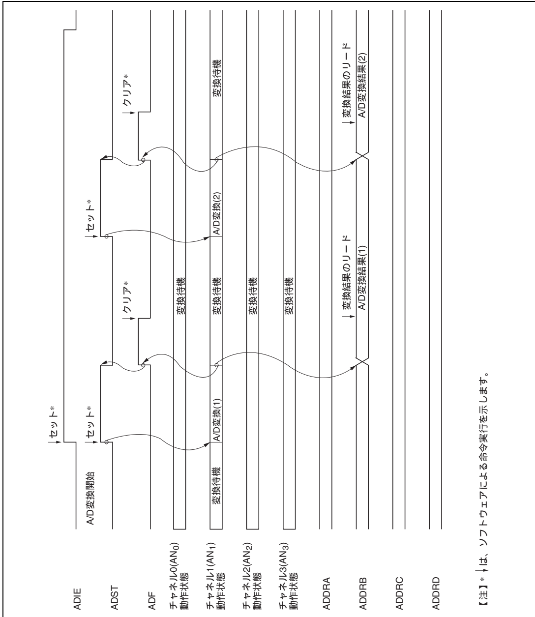
図 15.3 A/D 変換器の動作例 (単一モード チャンネル1 選択時)
