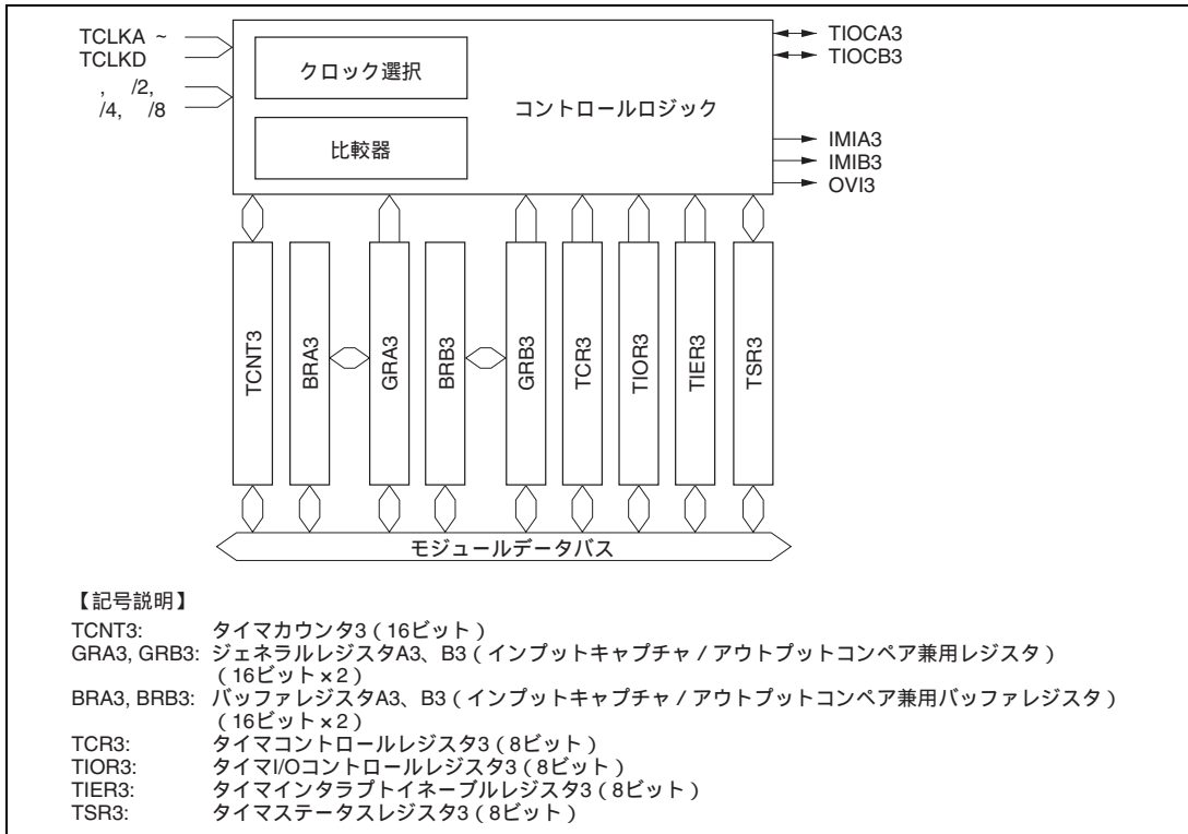
図 10.4 チャンネル3のブロック図
