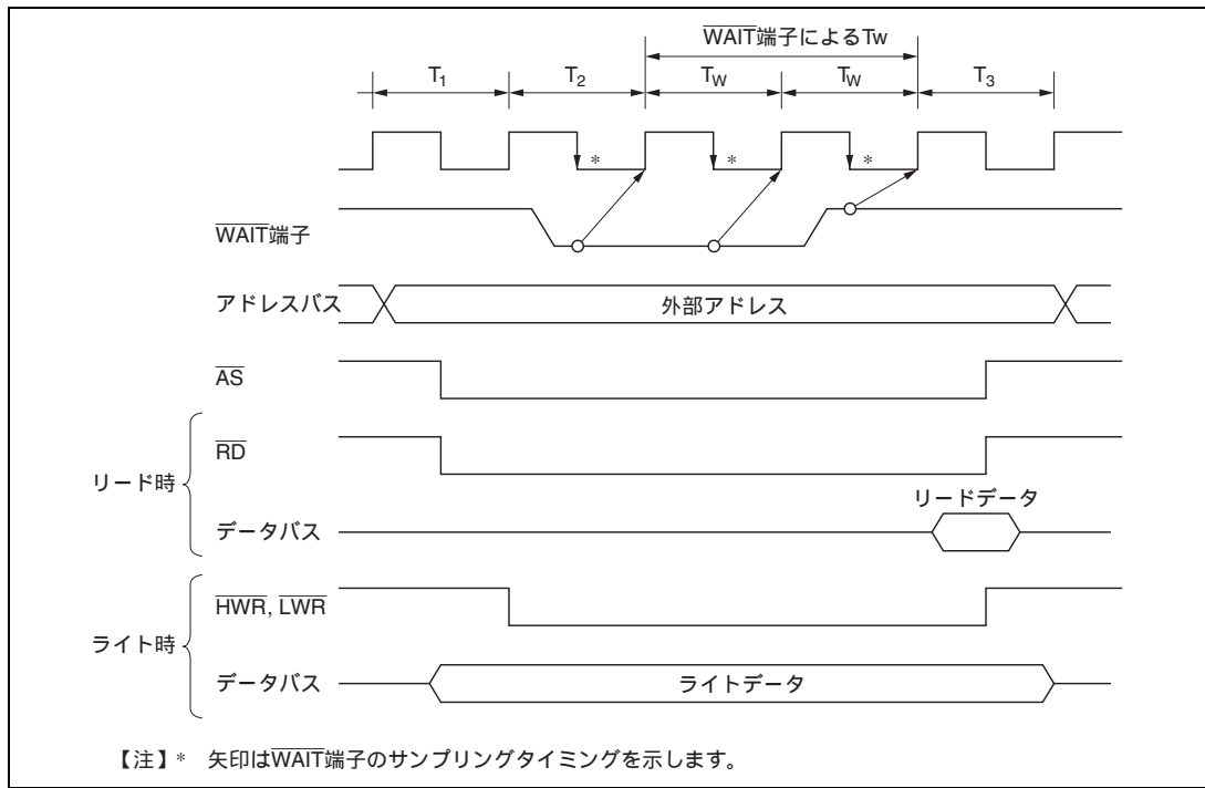
図 6.12 端子ウェイトモード 0
