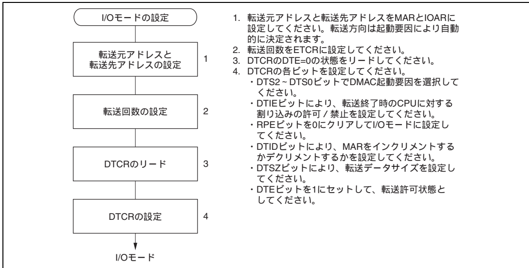
図 8.3 I/O モードの設定手順例
