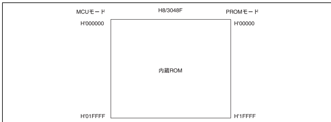
図 19.15 PROM モード時のメモリマップ
