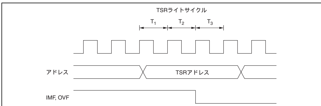
図 10.60 ステータスフラグのクリアタイミング
