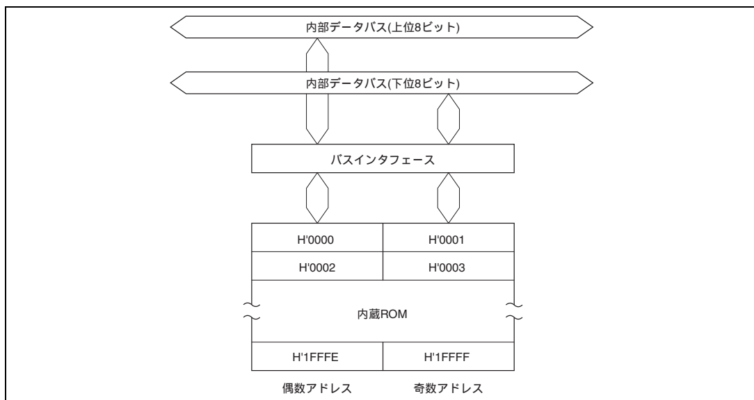
図 18.1 ROM のブロック図 (H8/3048、モード 7 の場合)
