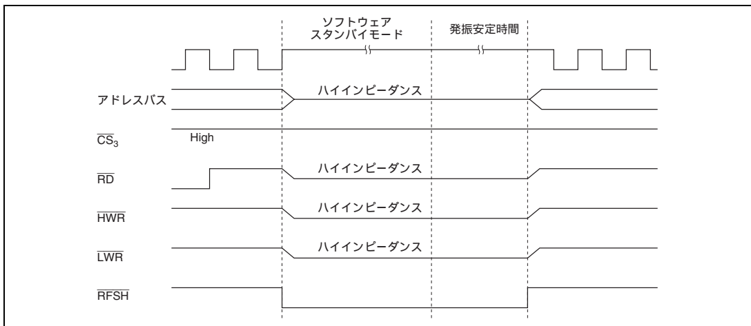
図 7.16 セルフリフレッシュモードの信号出力タイミング (PSRAME = 1、DRAME = 0)
