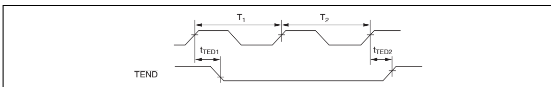
図 22.28 DMAC \overline{\text{TEND}} 出力タイミング / 2 ステートアクセス
