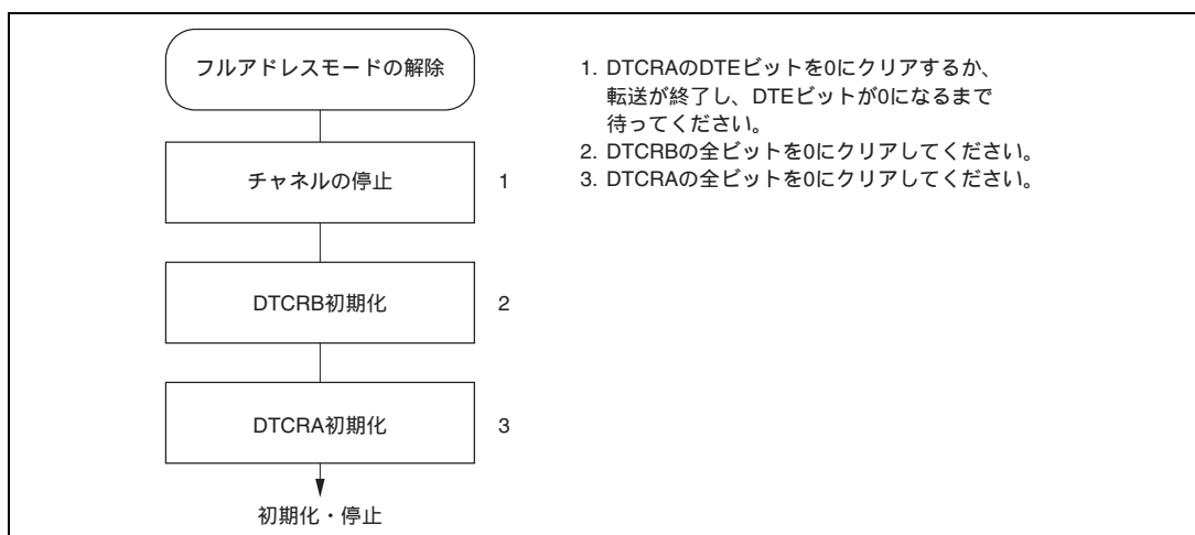
図 8.23 フルアドレスモードの解除手順例
