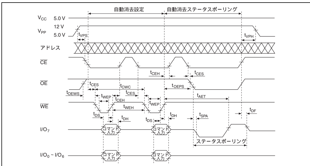
図 19.19 自動消去タイミング
