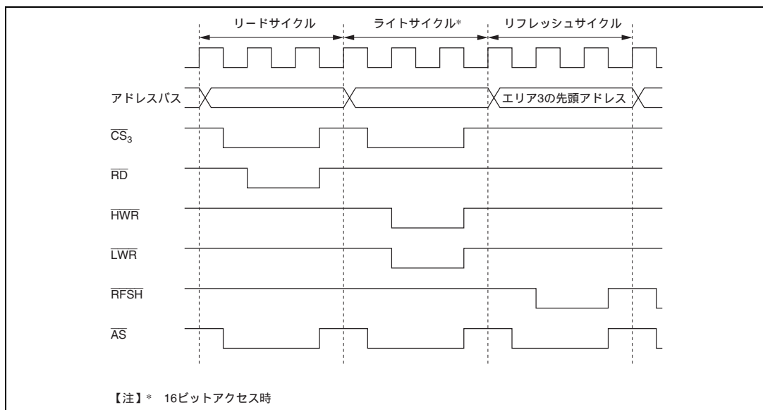
図 7.15 PSRAM 制御信号出力タイミング
