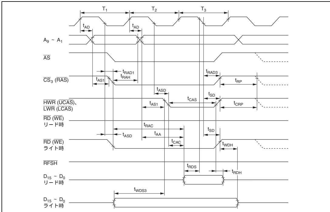
図 22.13 DRAM バスタイミング (リード/ライト時) / 3 ステートアクセス 2CAS 方式
