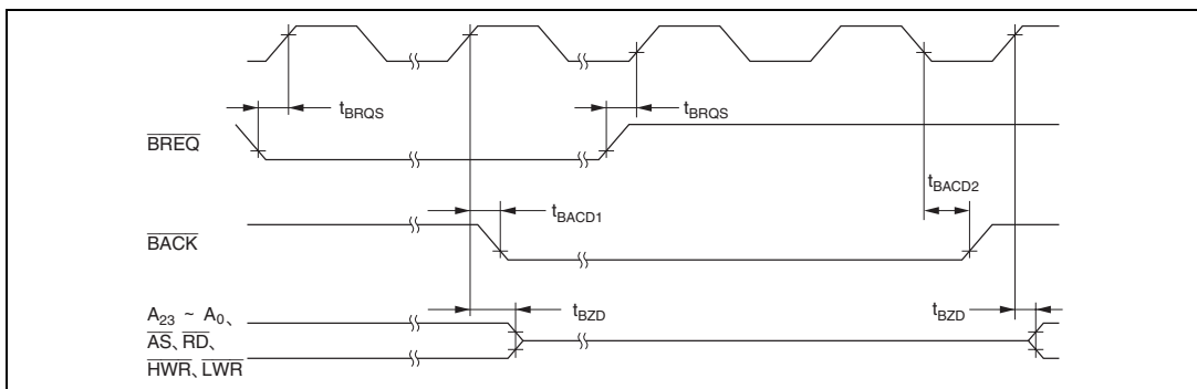
図 22.21 バスリリースモードタイミング
