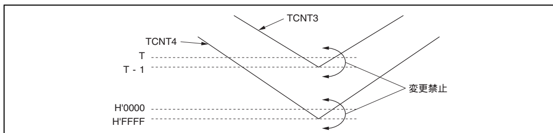
図 10.41 バッファ動作による GR の設定変更時の注意 (2)
