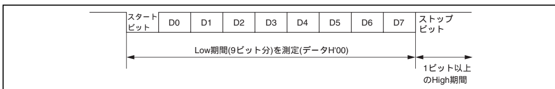
図 19.5 ホスト送信データの Low 期間の測定
