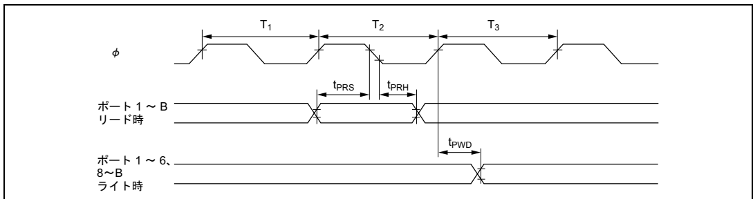
図 21.23 TPC、I/O ポート入出力タイミング
