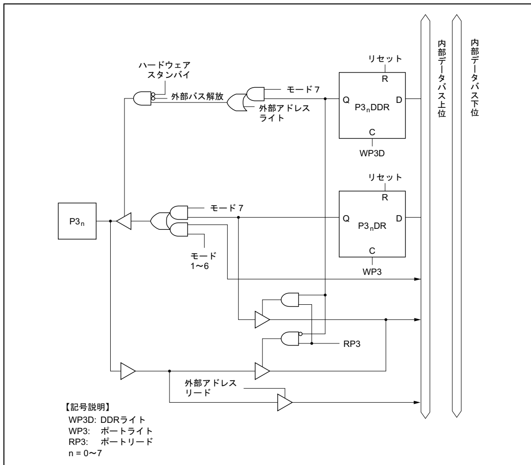
図 C.3 ポート3ブロック図 (P3 0 ~P3 7 端子)
