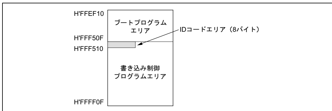
図 18.8 ブートモード時の RAM エリア
