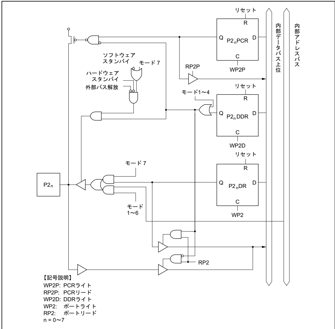
図 C.2 ポート2ブロック図 (P2 0 ~P2 7 端子)
