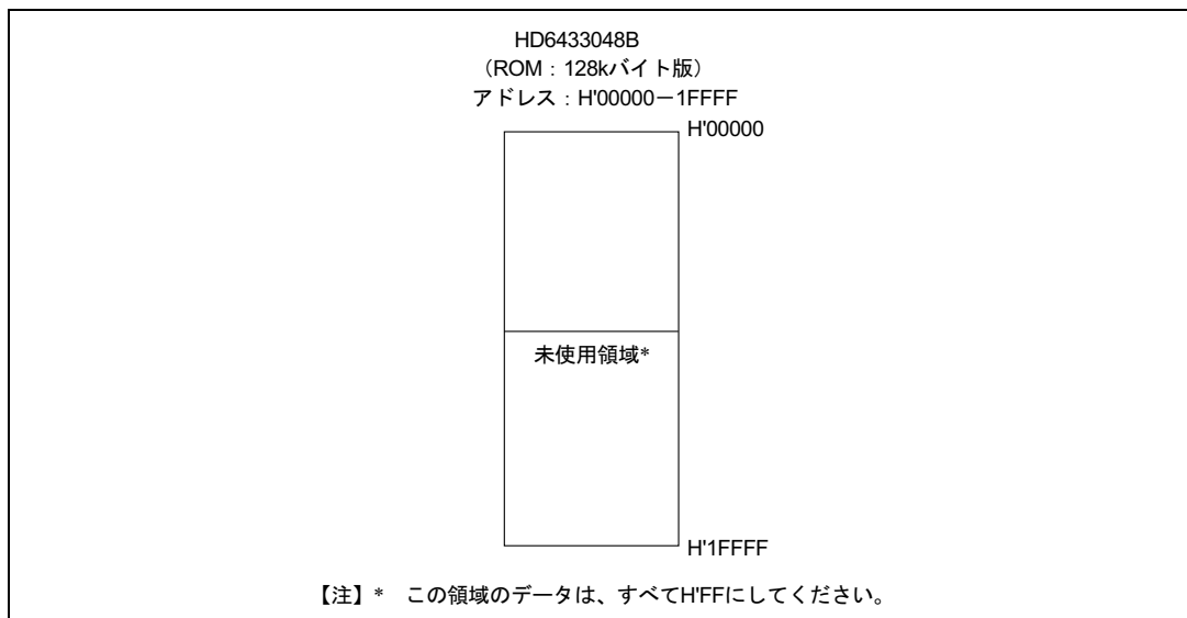
図 18.21 ROM アドレスとデータ
