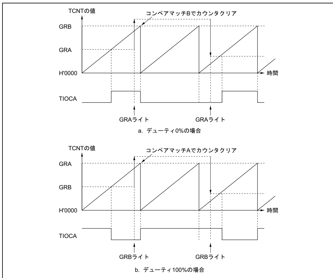
図 10.30 PWM モードの動作例 (2)
