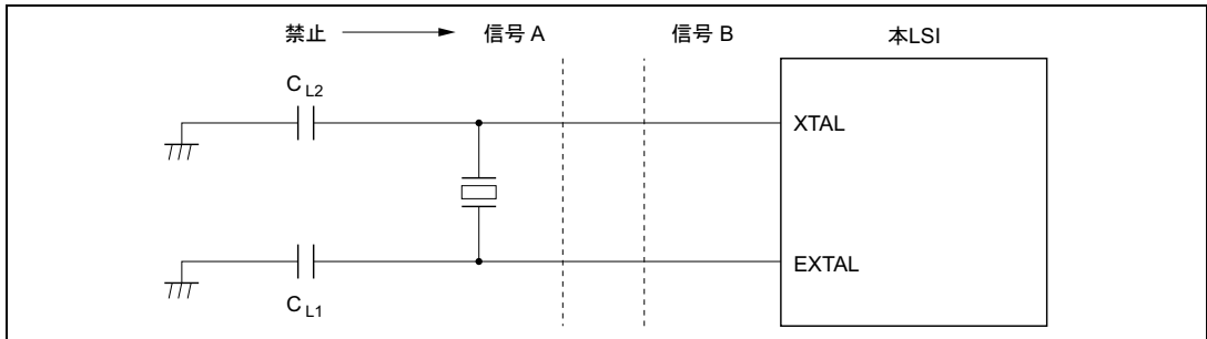
図 19.4 発振回路部のボード設計に関する注意事項
