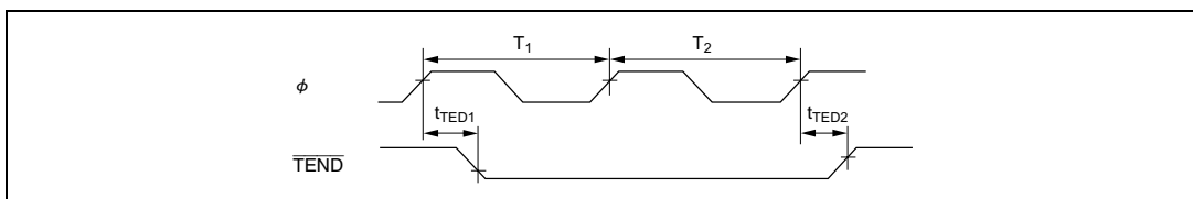
図 21.28 DMAC \overline{\text{TEND}} 出カタイミング / 2 ステートアクセス
