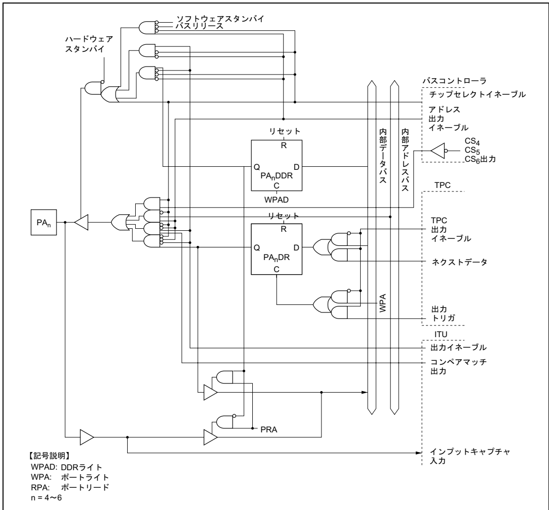
図 C.10 (c) ポート A ブロック図 (PA 4 ~PA 6 端子)
