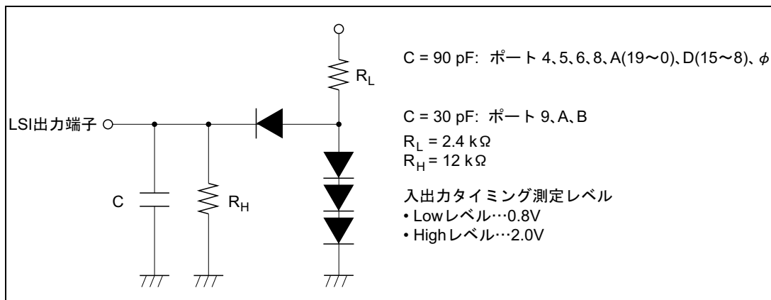
図 21.3 出力負荷回路
