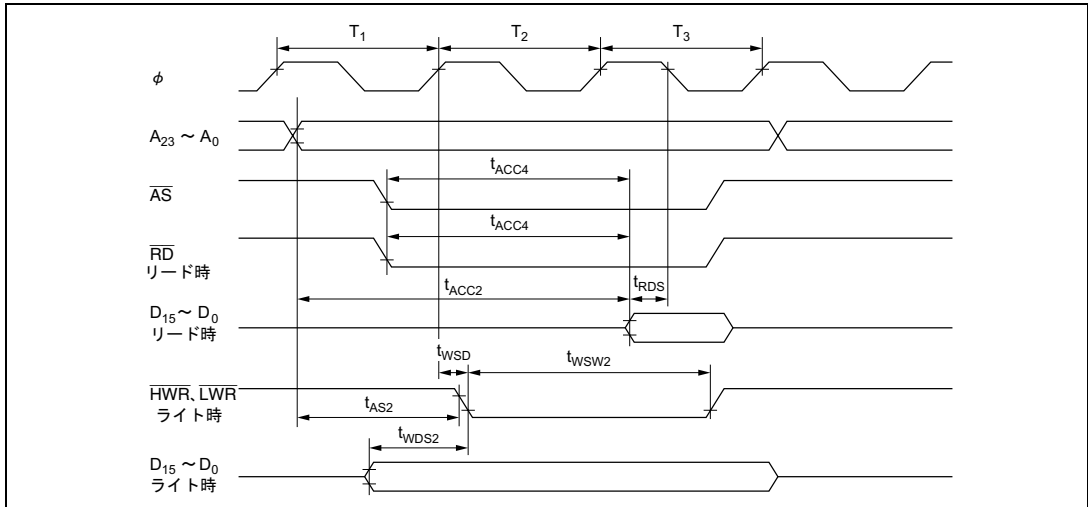
図 21.8 基本バスタイミング/3ステートアクセス
