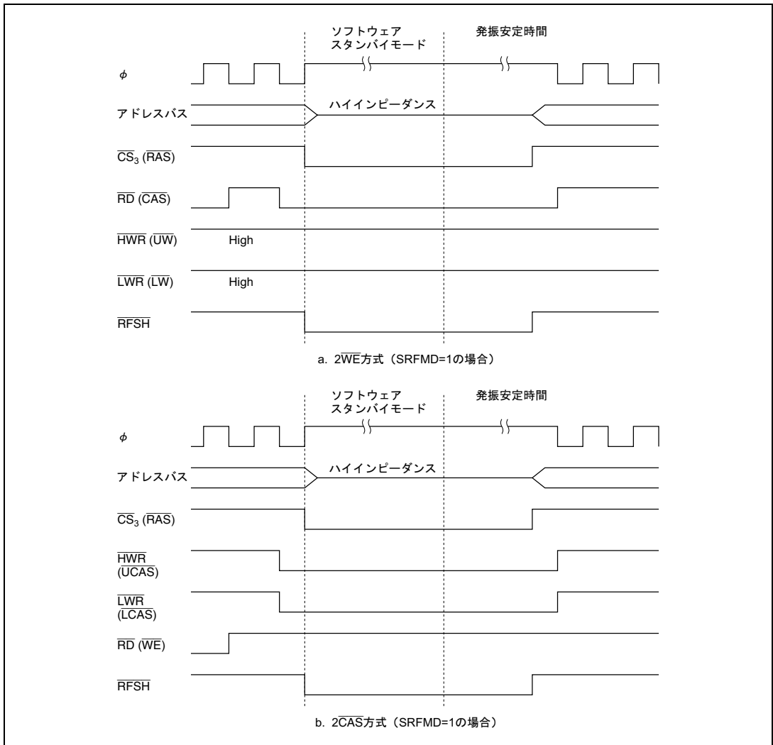
図 7.6 セルフリフレッシュモードの信号出力タイミング (PSRAM=0、DRAME=1)
