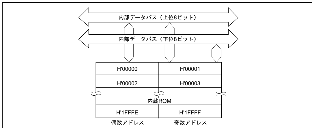
図 18.20 ROM のブロック図 (H8/3048B マスク ROM 品の場合)
