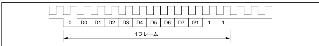
図 13.3 出カクロックと通信データの位相関係 (調歩同期式モード)
