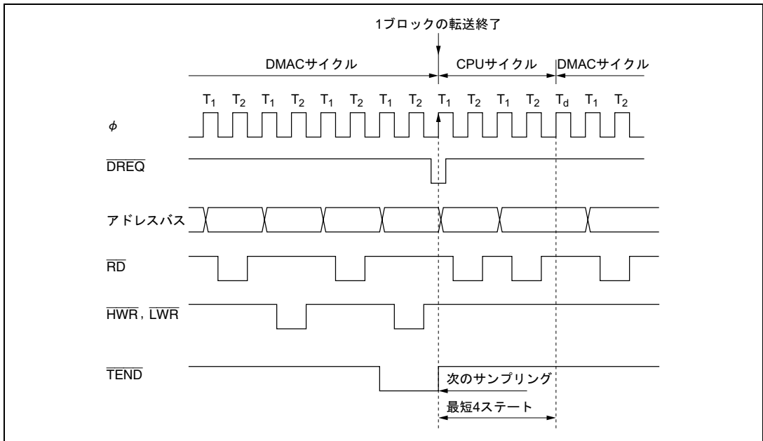
図 8.18 ブロック転送モード時の \overline{DREQ} 端子の立ち下がリエッジによる DMAC 起動タイミング
