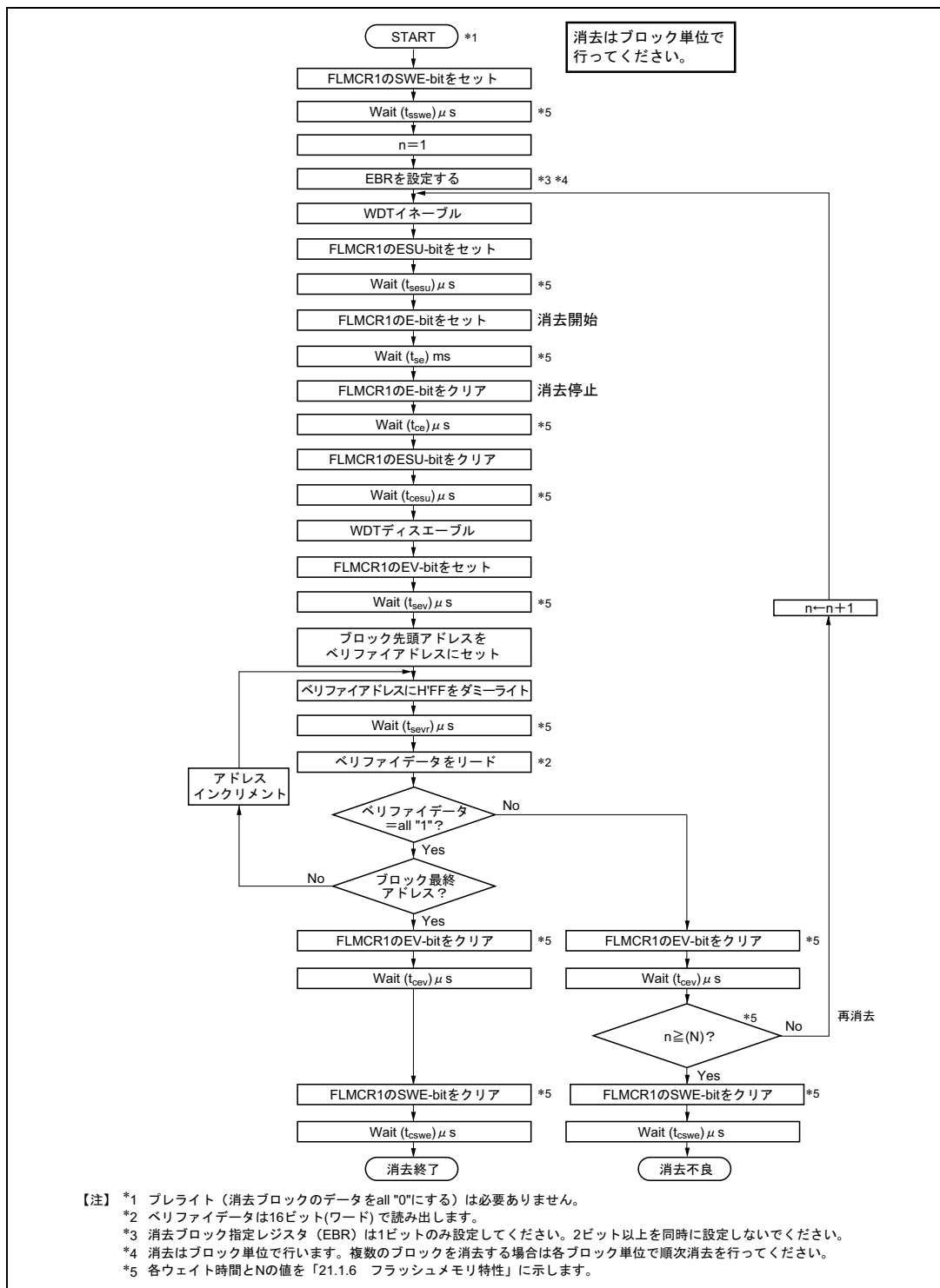
図 18.13 イレース/イレースペリファイフロー（単一ブロック消去）
