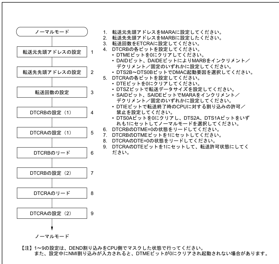
図 8.9 ノーマルモードの設定手順例
