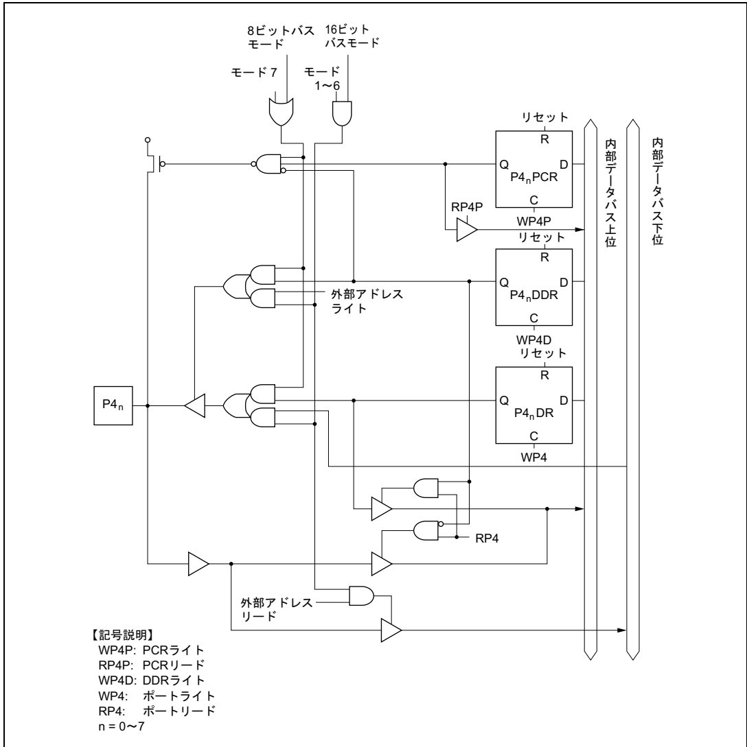
図 C.4 ポート4ブロック図 (P4 0 ~P4 7 端子)
