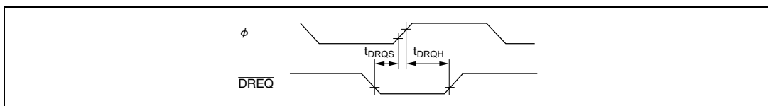
図 21.30 DMAC \overline{\text{DREQ}} 入カタイミング
