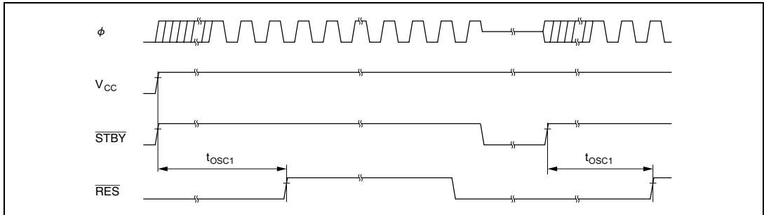
図 21.22 発振安定時間タイミング
