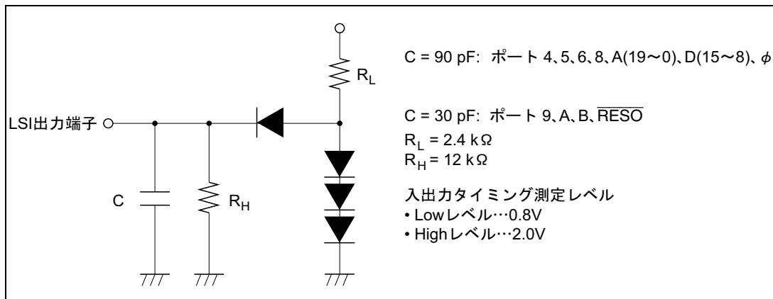
図 21.6 出力負荷回路
