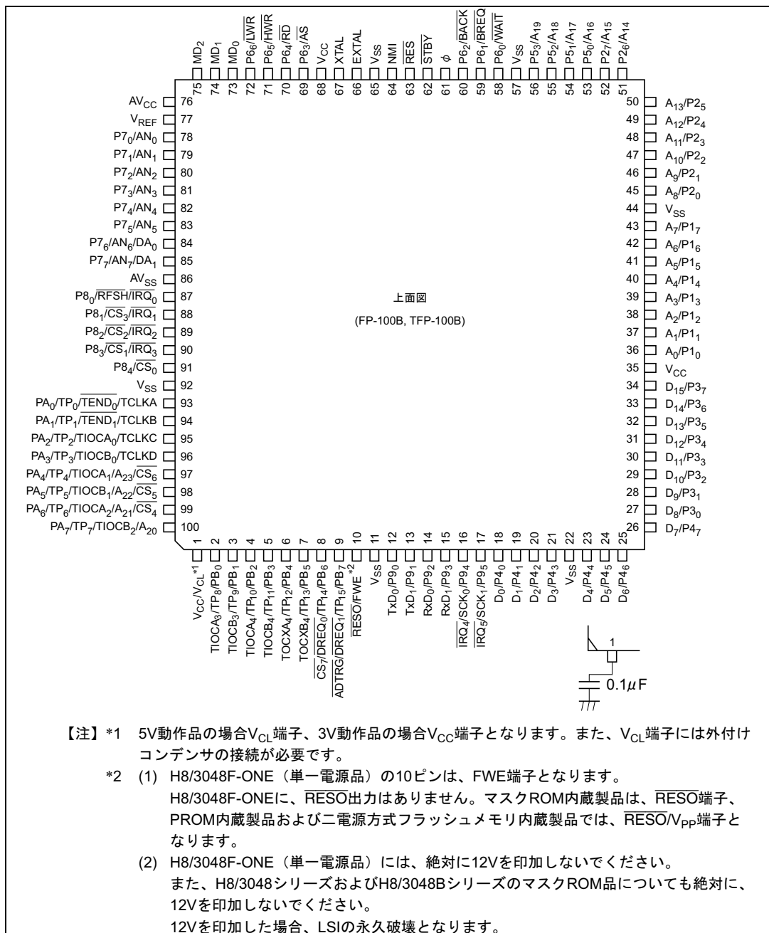
図 1.3 H8/3048B シリーズピン配置図 (FP-100B、TFP-100B : 上面図)
