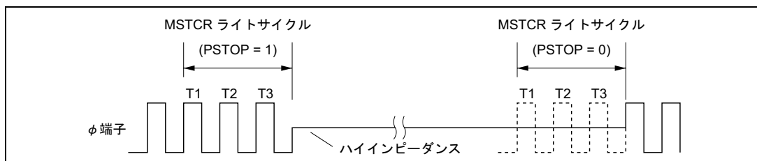
図 20.3 \phi クロック発振開始、発振停止タイミング
