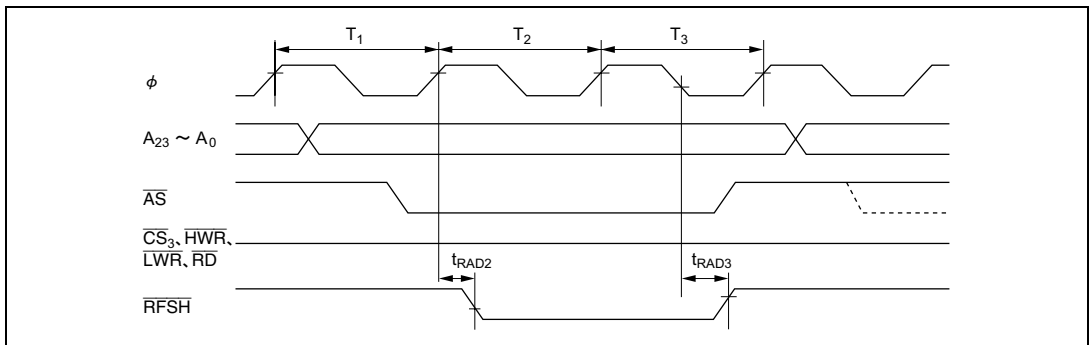
図 21.17 PSRAM バスタイミング (リフレッシュサイクル時) /3 ステートアクセス
