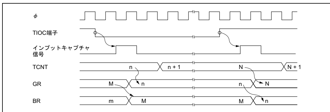
図 10.52 バッファ動作時の入力キャプチャタイミング
