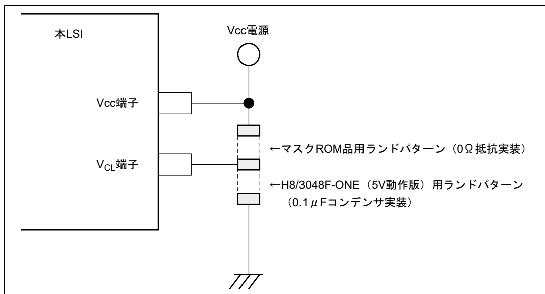
図 1.6 外付けコンデンサ対応の基板パターン例
