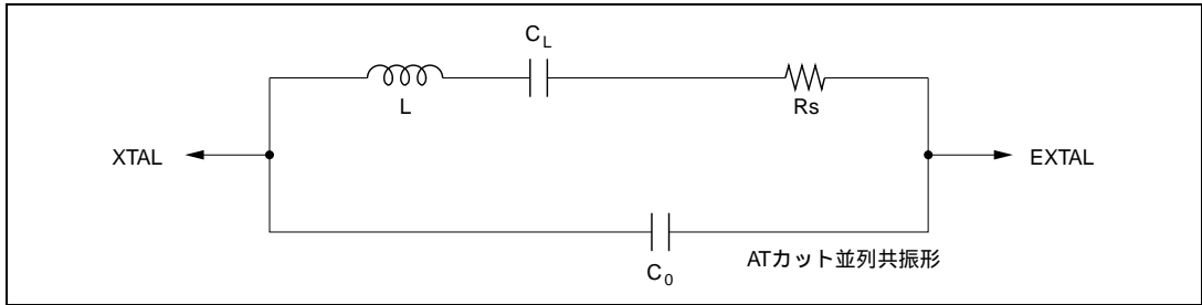
図 19.3 水晶発振子の等価回路
