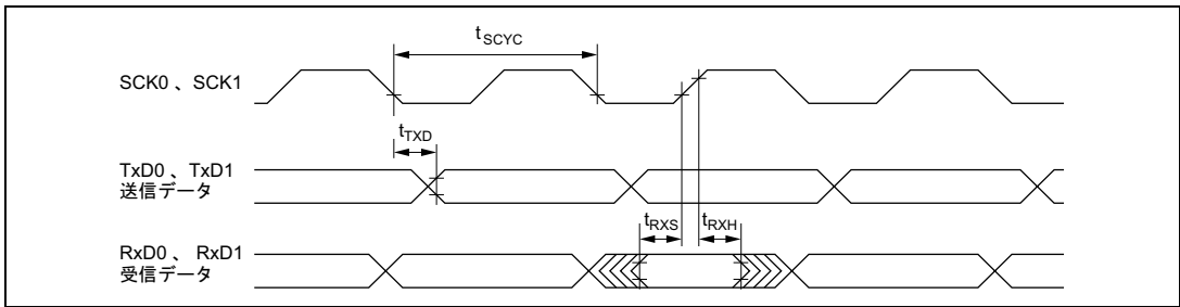
図 21.27 クロック同期式モード時の SCI 入出力タイミング
