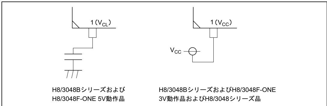
図 1.2 1 ピンの接続図
