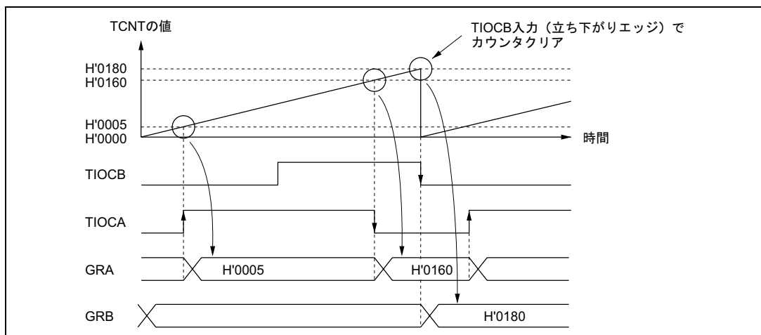
図 10.24 インพุットキャプチャ動作例
