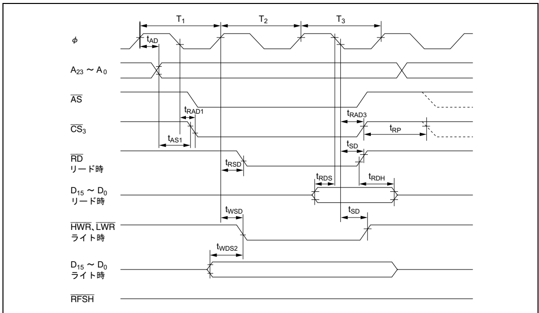
図 21.16 PSRAM バスタイミング (リード/ライト時) /3 ステートアクセス
