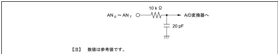
図 15.8 アナログ入力端子等価回路
