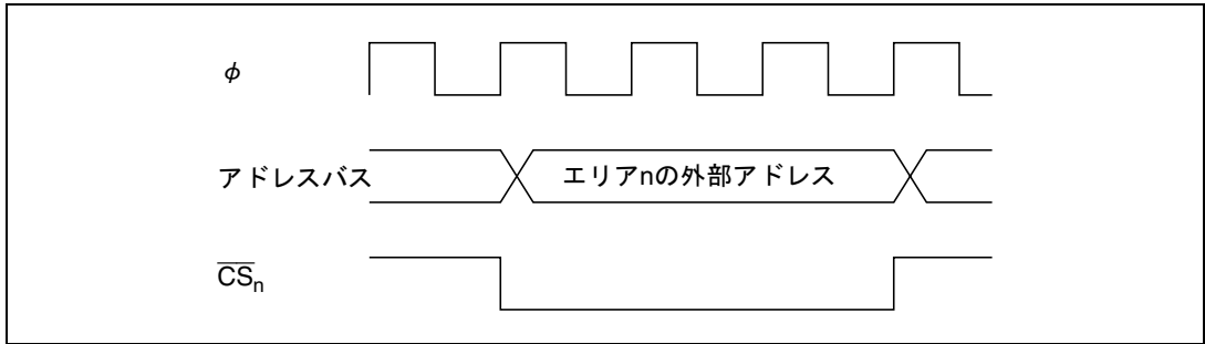
図 6.3 \overline{CS}_n 信号の出力タイミング (n=7~0)
