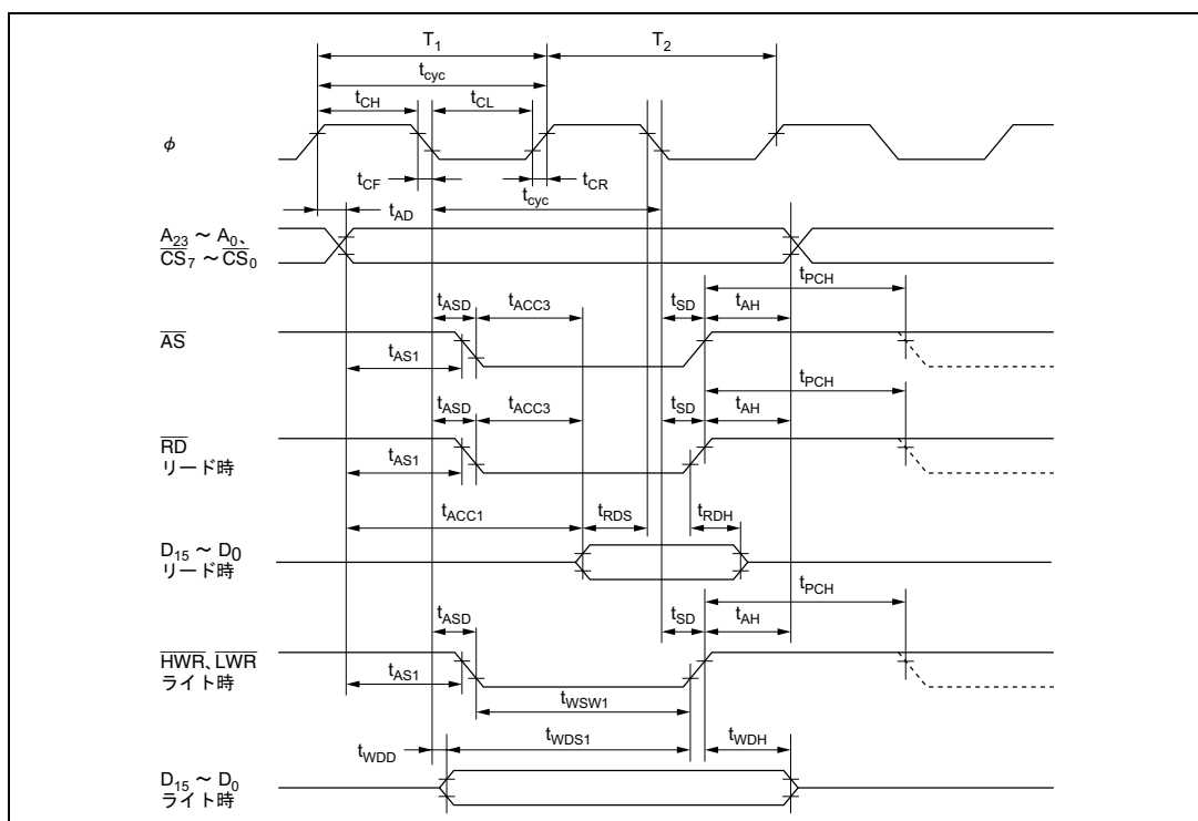
図 21.7 基本バスタイミング/2ステートアクセス
