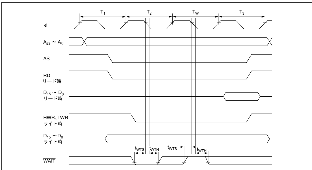
図 21.9 基本バスタイミング/3ステートアクセス1ウェイト
