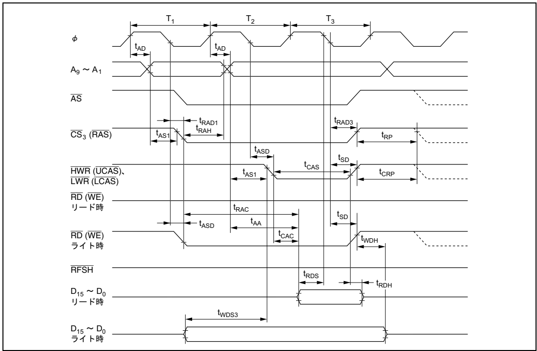
図 21.13 DRAM バスタイミング (リード/ライト時) /3 ステートアクセス — 2CAS 方式 —
