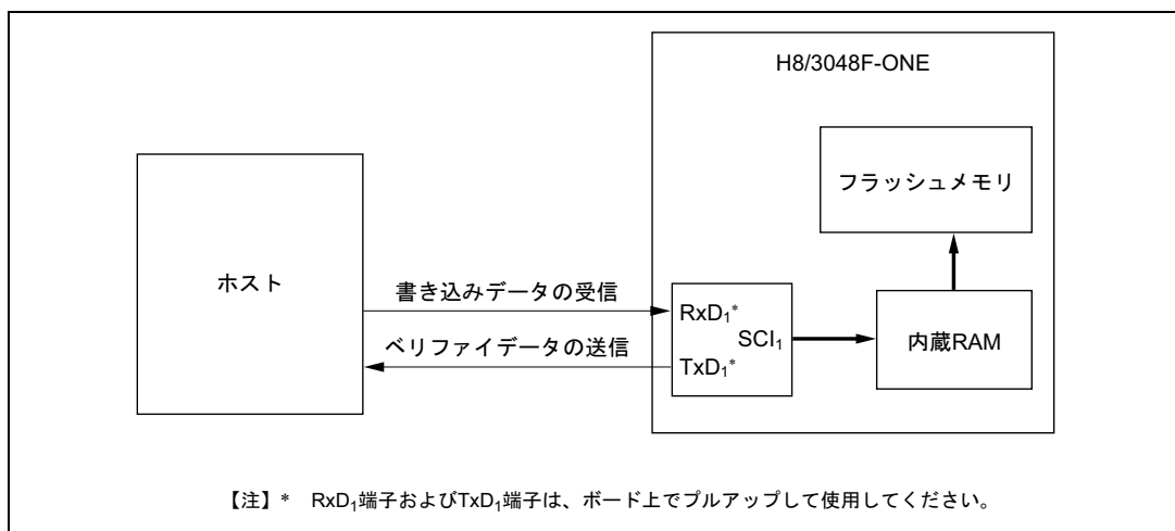
図 18.6 ブートモード時のシステム構成図
