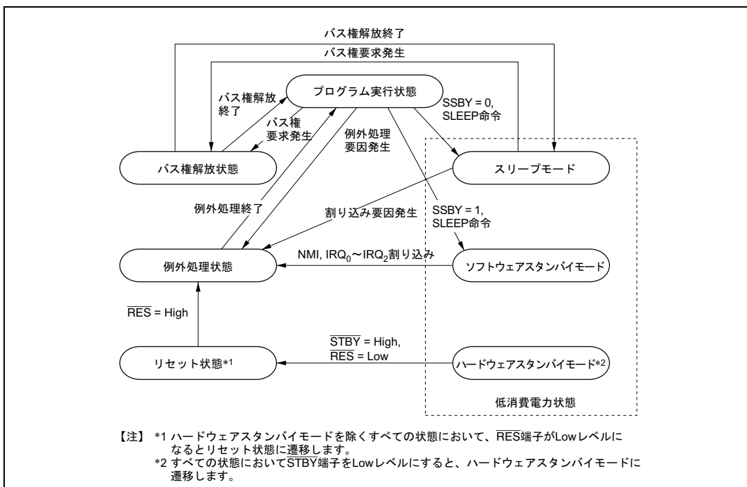
図 2.13 状態遷移図
