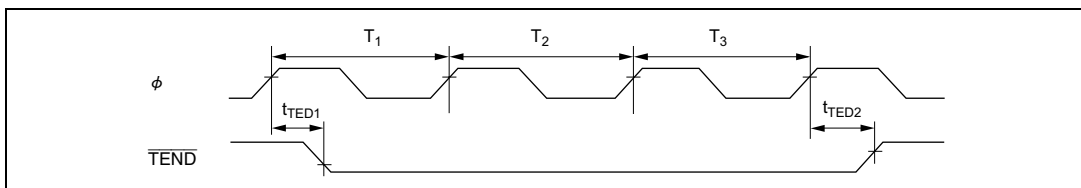
図 21.29 DMAC \overline{\text{TEND}} 出カタイミング / 3 ステートアクセス
