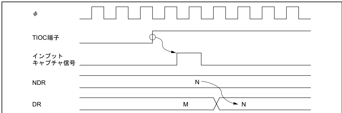
図 11.8 インพุットキャプチャによる TPC 出力例
