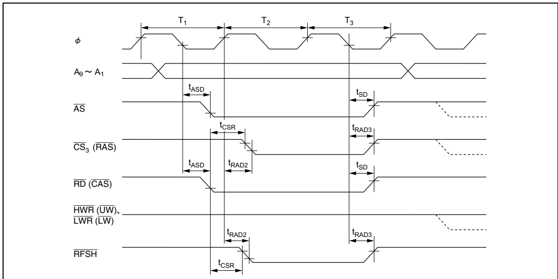
図 21.11 DRAM バスタイミング (リフレッシュサイクル時) /3 ステートアクセス — 2WE 方式 —
