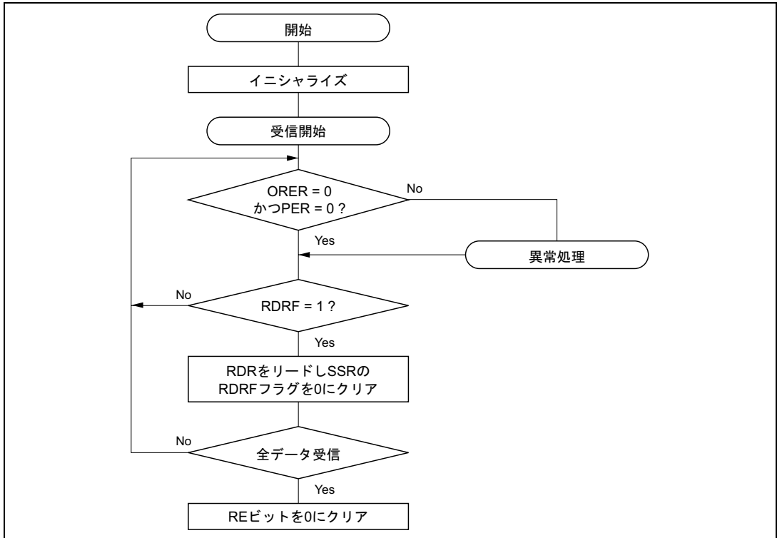
図 14.7 受信処理フローの例
