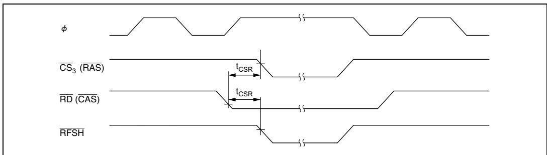
図 21.12 DRAM バスタイミング (セルフリフレッシュモード) — 2WE 方式 —
