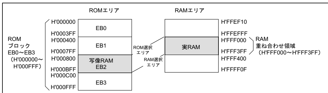
図 18.5 ROM エリアと RAM エリアの重ね合わせ例
