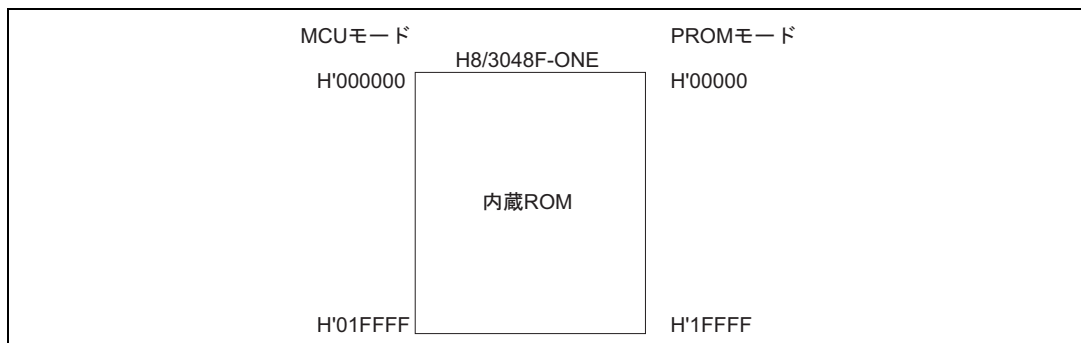
図 18.16 PROM モード時のメモリマップ
