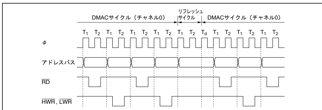
図 8.20 リフレッシュコントローラと DMAC の動作タイミング
