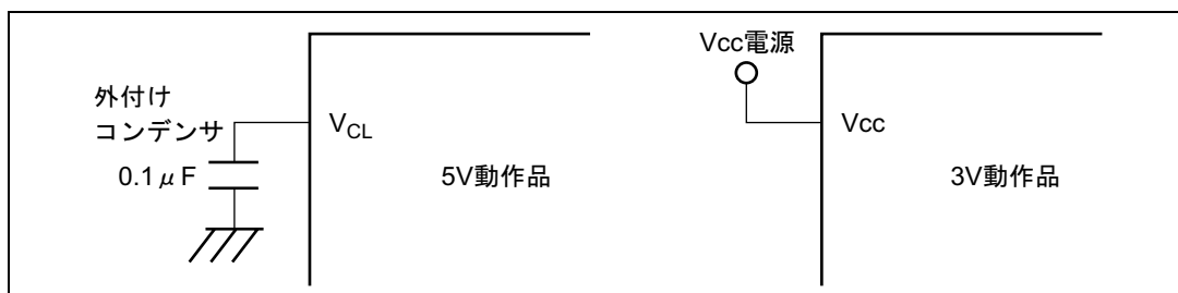
図 1.5 5V 動作品と 3V 動作品との違い
