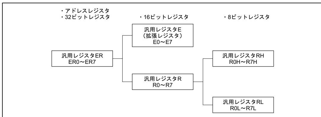
図 2.4 汎用レジスタの使用法
