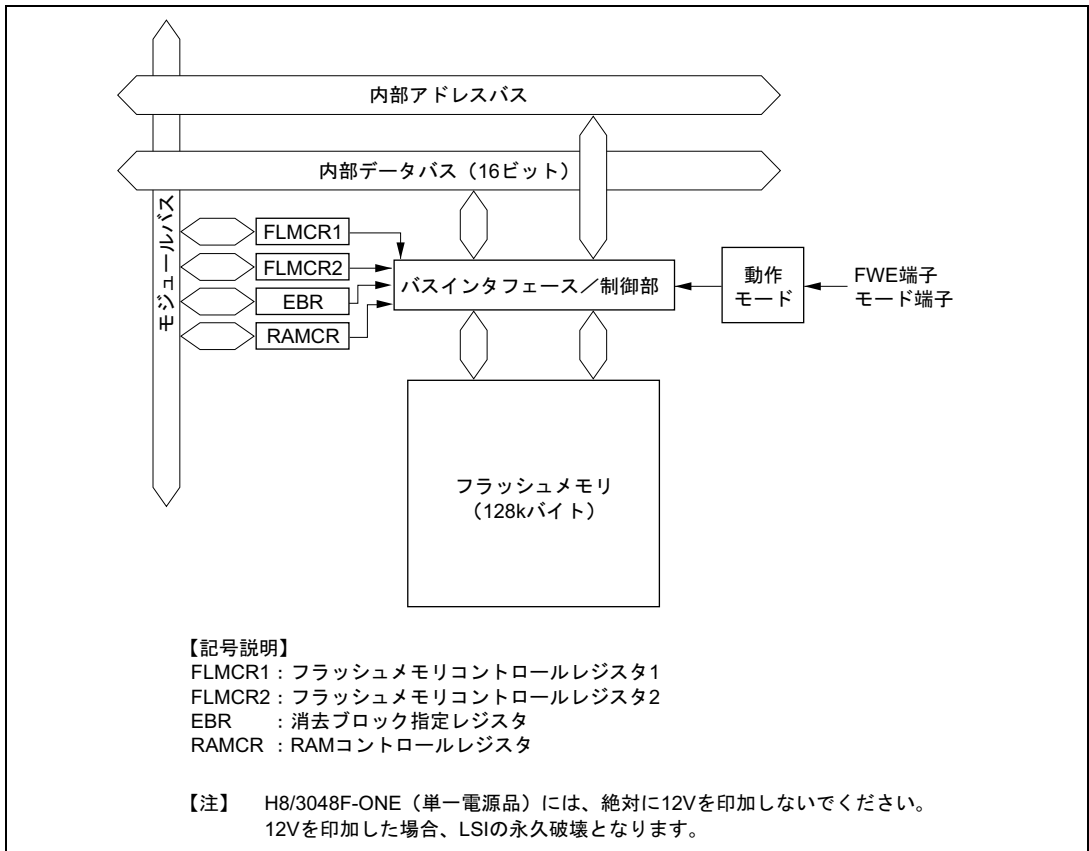
図 18.1 フラッシュメモリのブロック図
