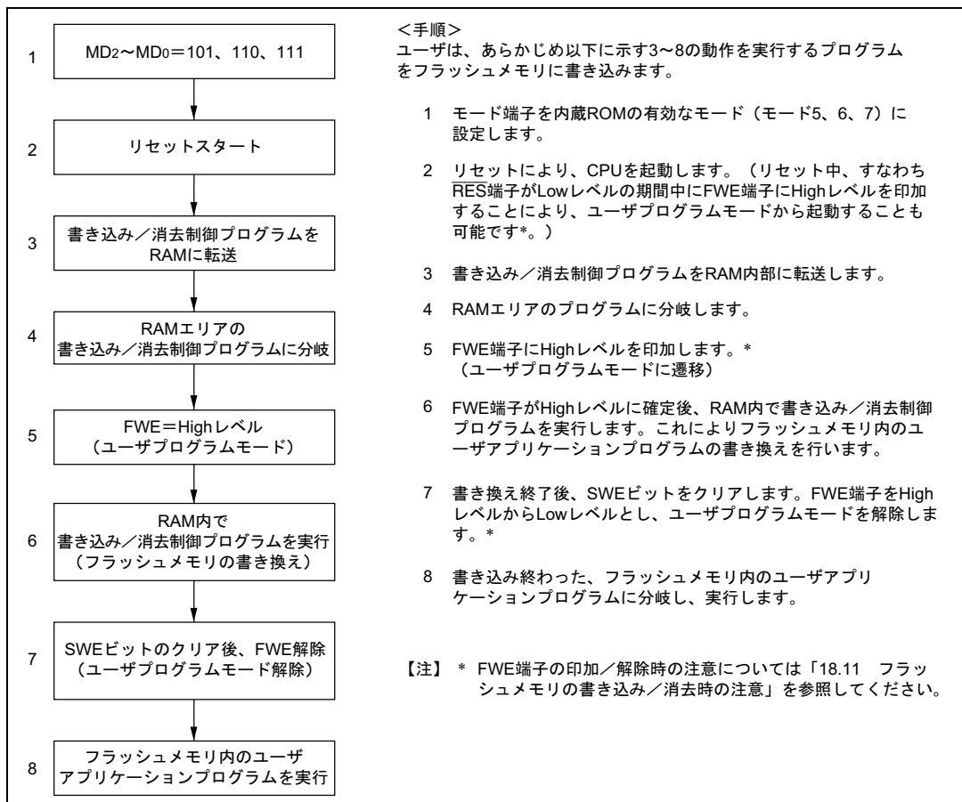
図 18.10 ユーザプログラムモードの実行手順例
