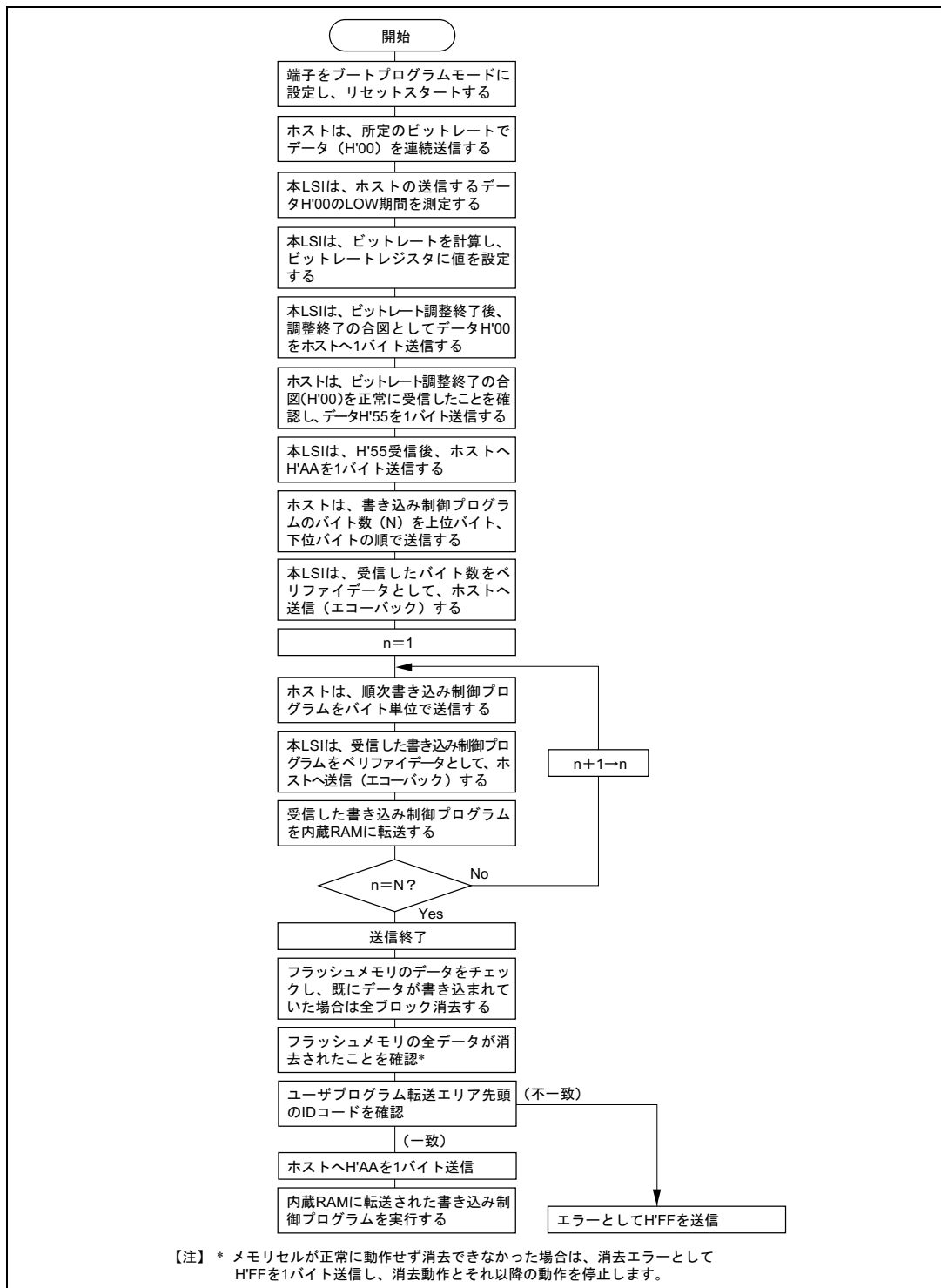
図 18.7 ブートモード実行手順
