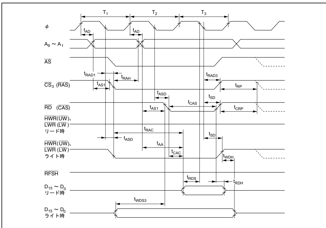
図 21.10 DRAM バスタイミング (リード/ライト時) /3 ステートアクセス — 2WE 方式 —
