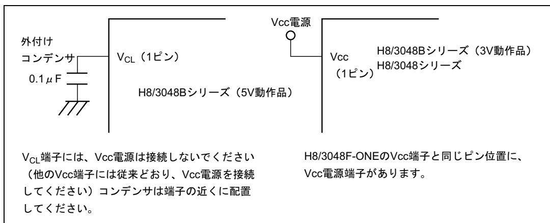
図 1.4 H8/3048B シリーズの V_{CL} コンデンサ接続方法
