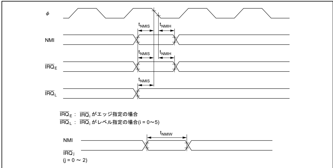
図 21.20 割り込み入力タイミング
