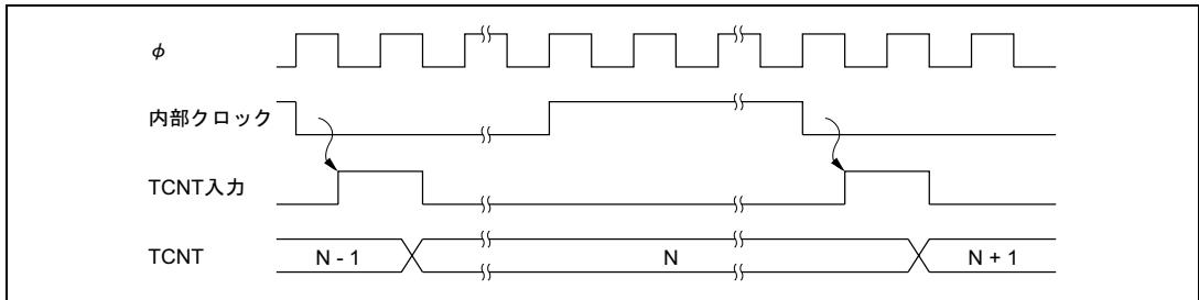
図 10.17 内部クロック動作時のカウンタタイミング
