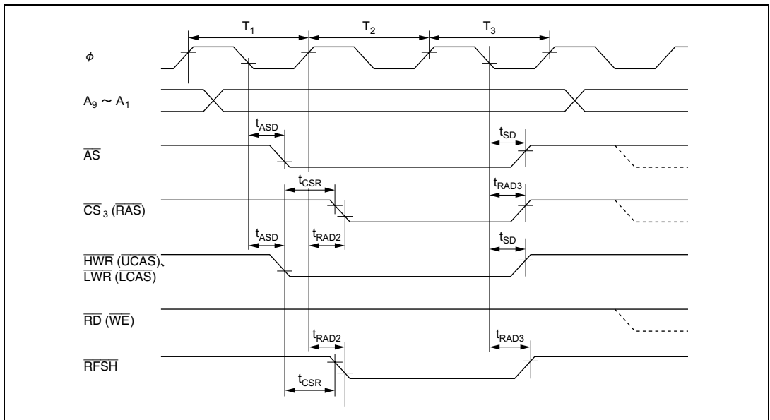
図 21.14 DRAM バスタイミング (リフレッシュサイクル時) /3 ステートアクセス — 2CAS 方式 —
