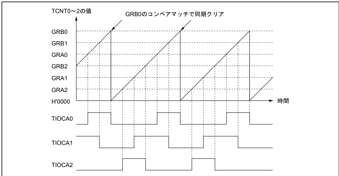
図 10.27 同期動作例
