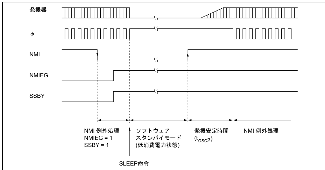
図 20.1 ソフトウェアスタンバイモード時の NMI タイミング (例)
