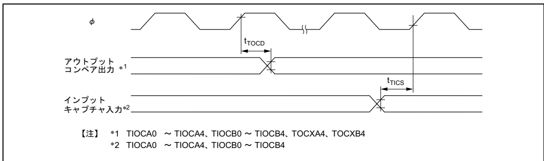
図 21.24 ITU 入出力タイミング
