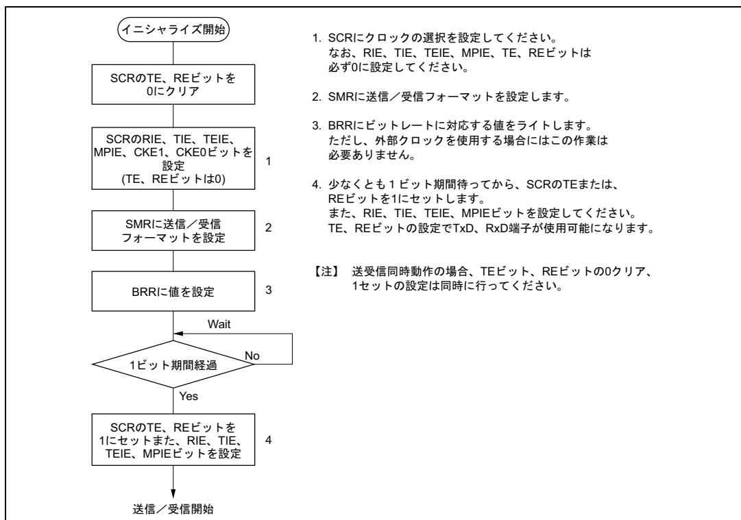
図 13.15 SCI のイニシャライズフローチャートの例
