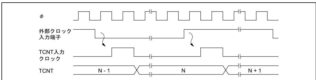
図 10.18 外部クロック動作時のカウンタタイミング (両エッジ検出の場合)
