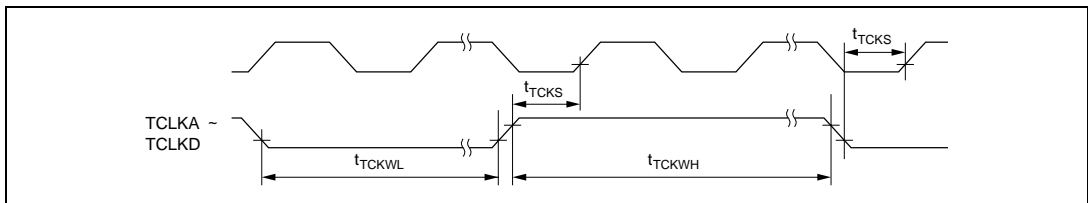
図 21.25 ITU 外部クロック入力タイミング
