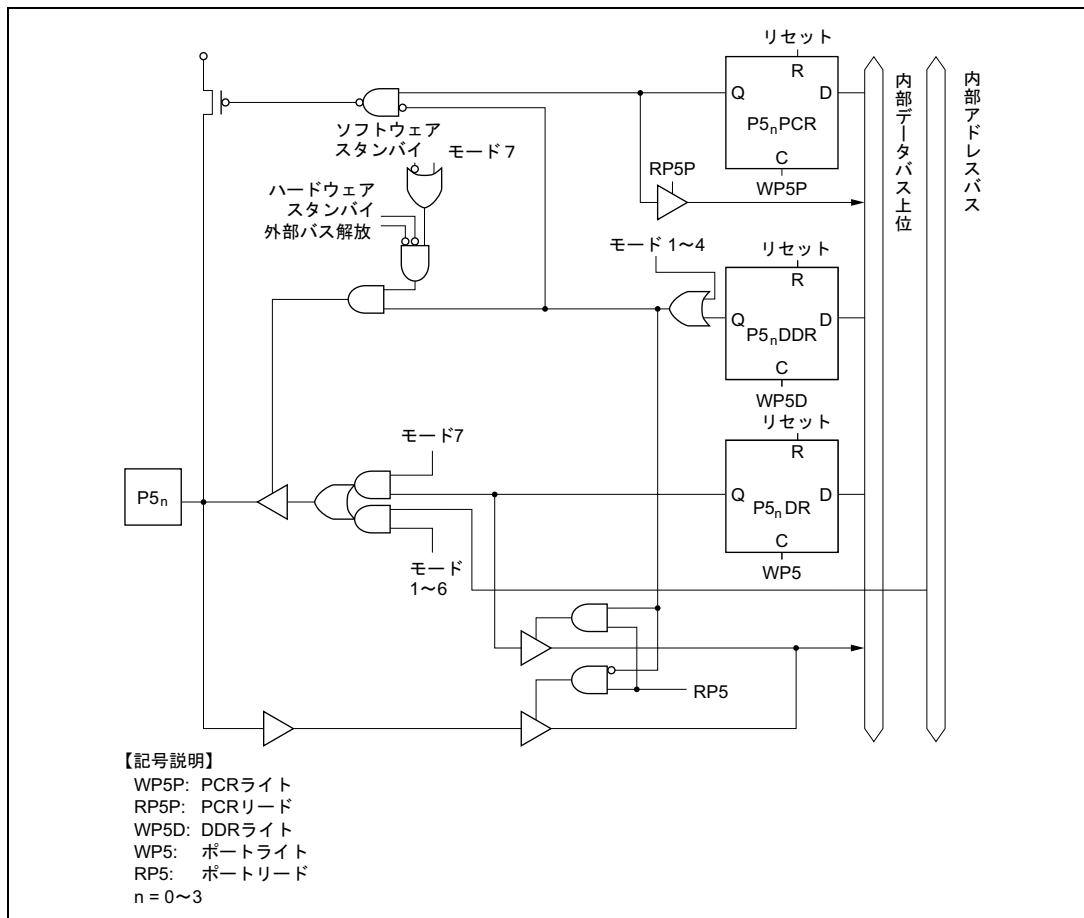
図 C.5 ポート5 ブロック図 (P5 0 ~P5 7 端子)
