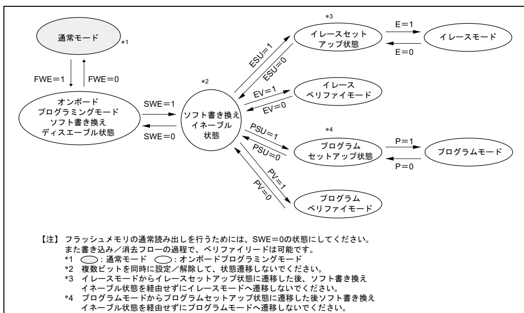
図 18.11 FLMCR1 の各ビット設定による状態遷移
