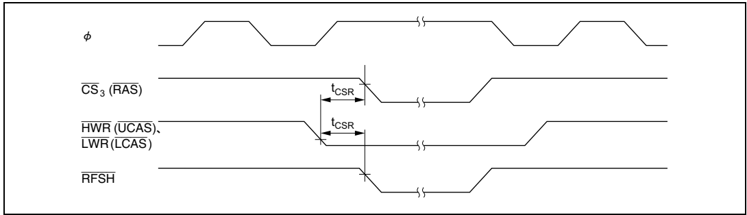
図 21.15 DRAM バスタイミング (セルフリフレッシュモード) — 2CAS 方式 —
