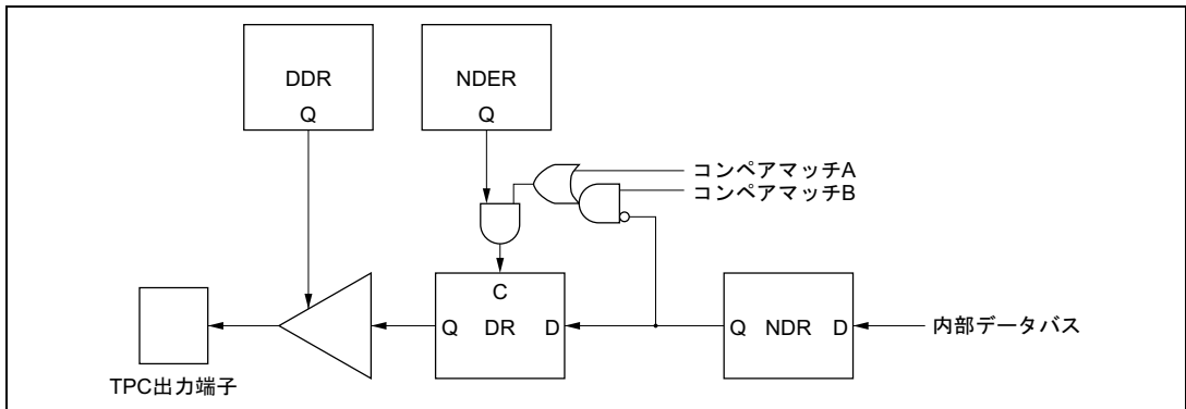
図 11.9 TPC 出力ノンオーバーラップ動作
