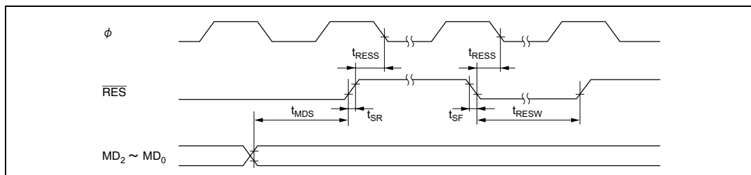
図 21.18 リセット入力タイミング
