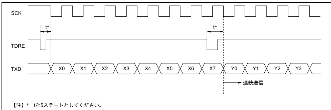
図 13.22 クロック同期式送信の例
