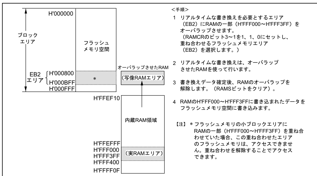
図 18.15 RAMのオーバーラップ動作例
