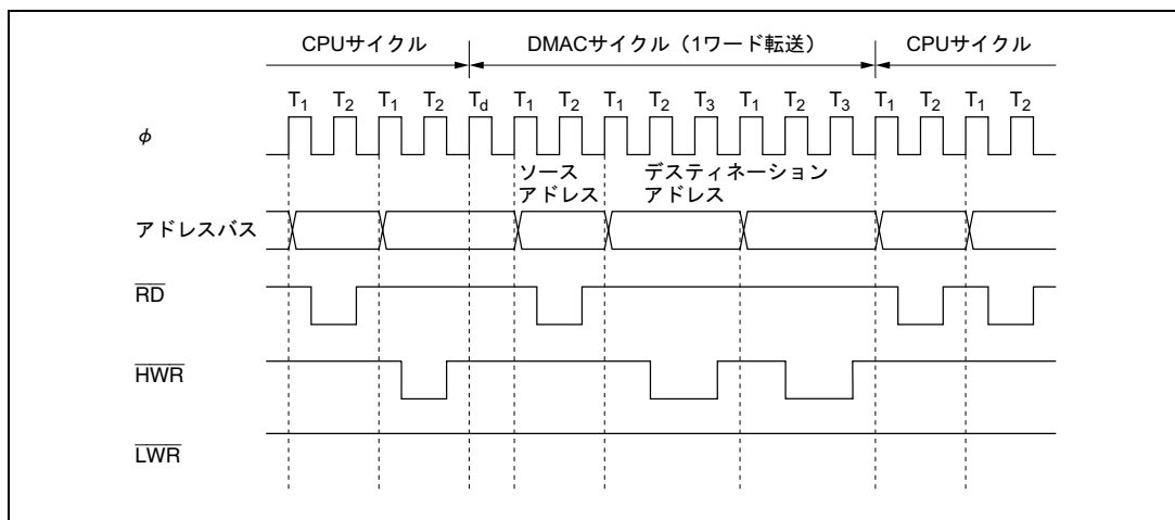
図 8.13 DMA 転送バスタイミング例
