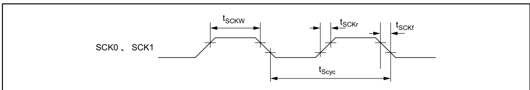
図 21.26 SCK 入力クロックタイミング
