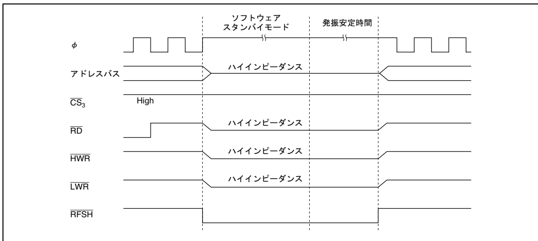
図 7.16 セルフリフレッシュモードの信号出力タイミング (PSRAM=1、DRAME=0)
