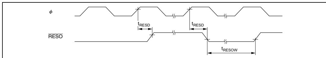
図 21.19 リセット出力タイミング*
