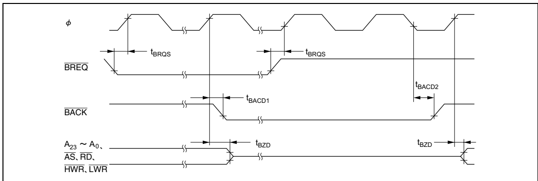
図 21.21 バスリリースモードタイミング
