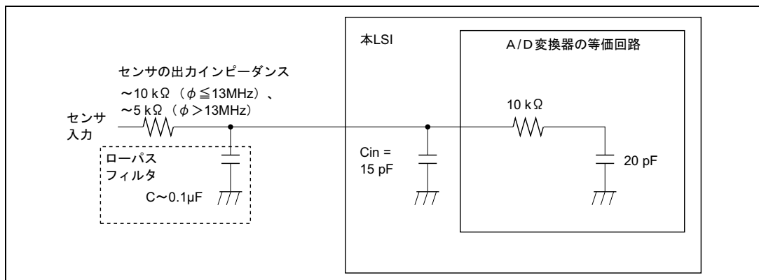
図 15.11 アナログ入力回路の例
