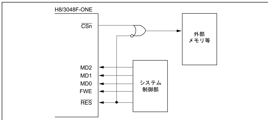
図 18.9 推奨システムブロック図
