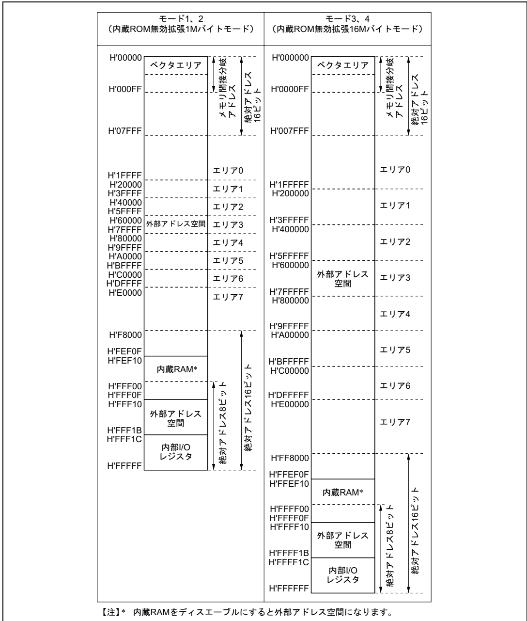
図 3.1 H8/3048B シリーズの各動作モードにおけるメモリマップ (1)
