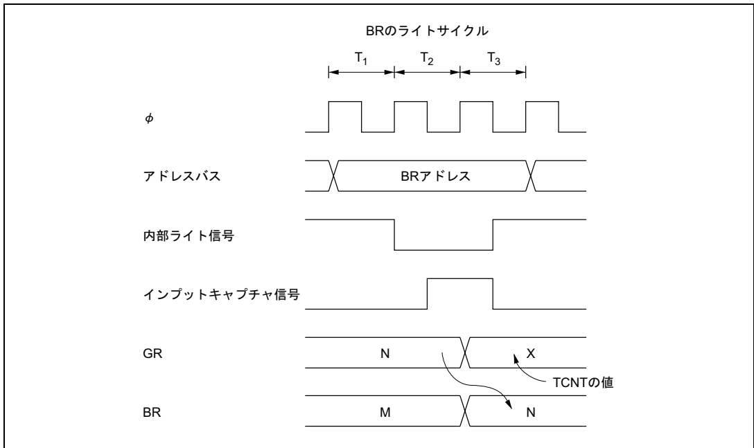
図 10.69 BR のライトと入力キャプチャの競合
