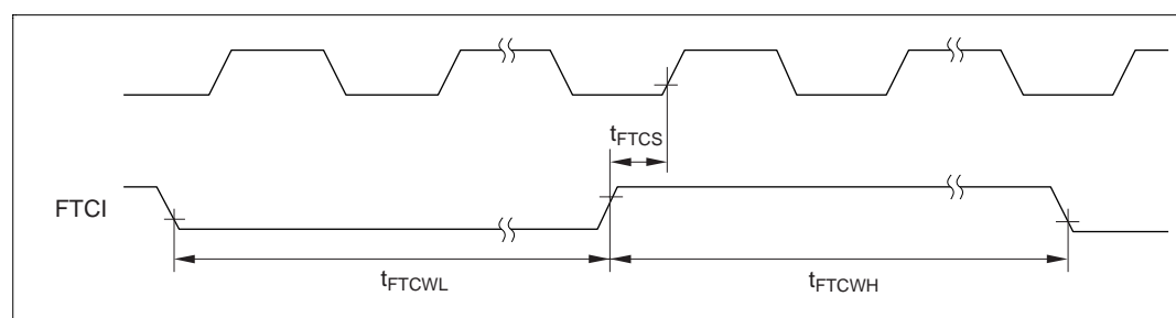
図 23.14 フリーランニングタイマ外部クロック入力タイミング
