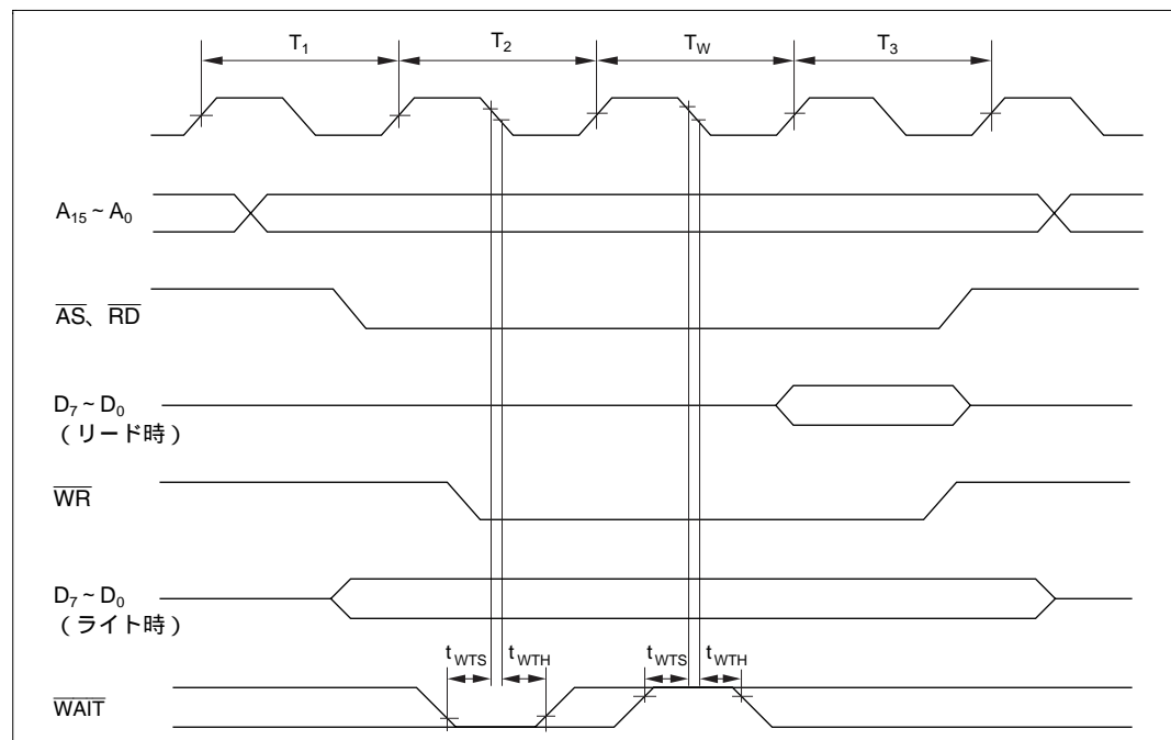
図 23.8 拡張モード (モード 1、2) 時基本バスサイクル (1 ウェイトステート)
