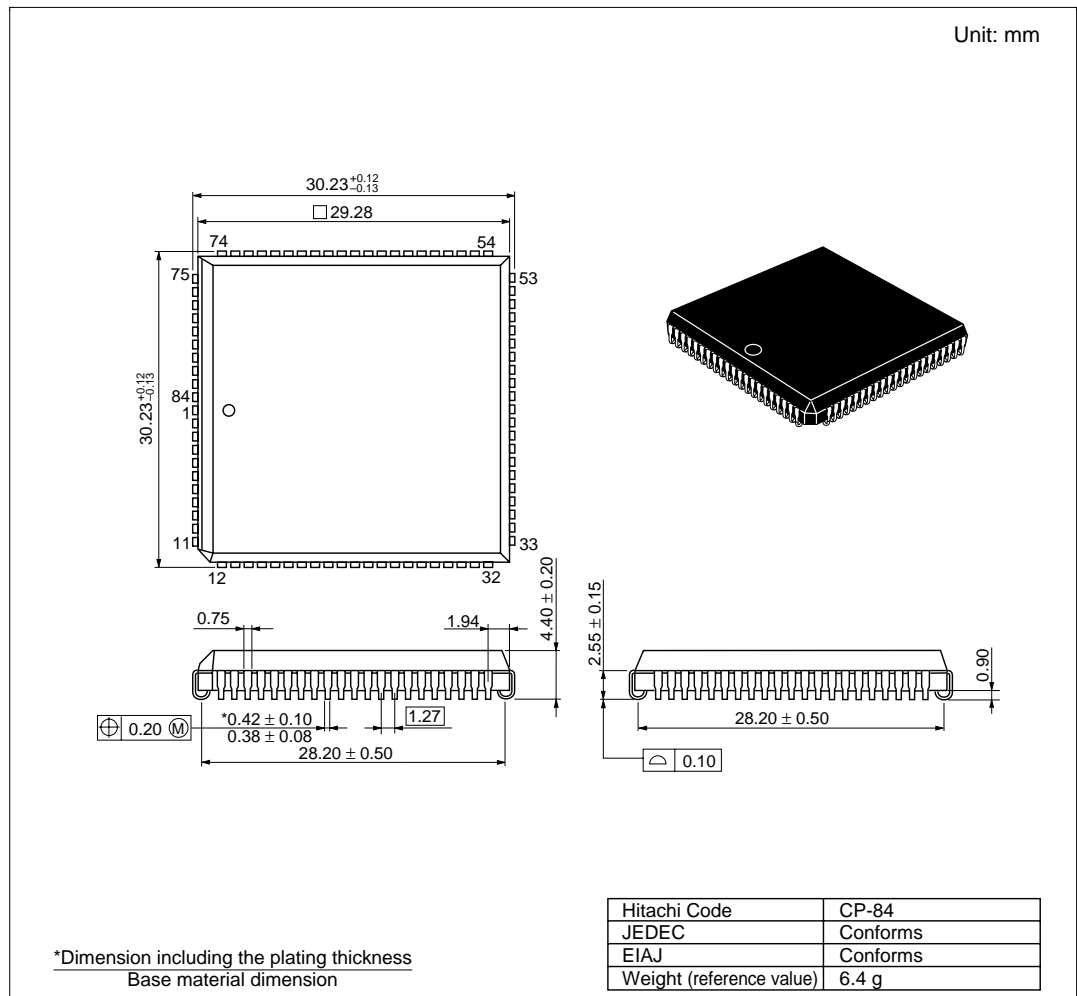
図 I.3 外形寸法図 (CP-84)
