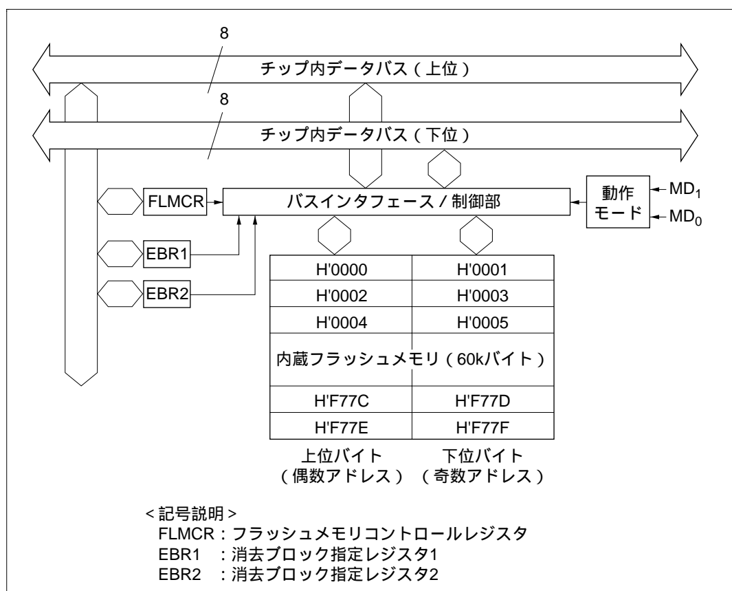
図 20.1 フラッシュメモリのブロック図
