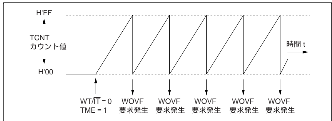
図 11.4 インターバルタイマモード時の動作
