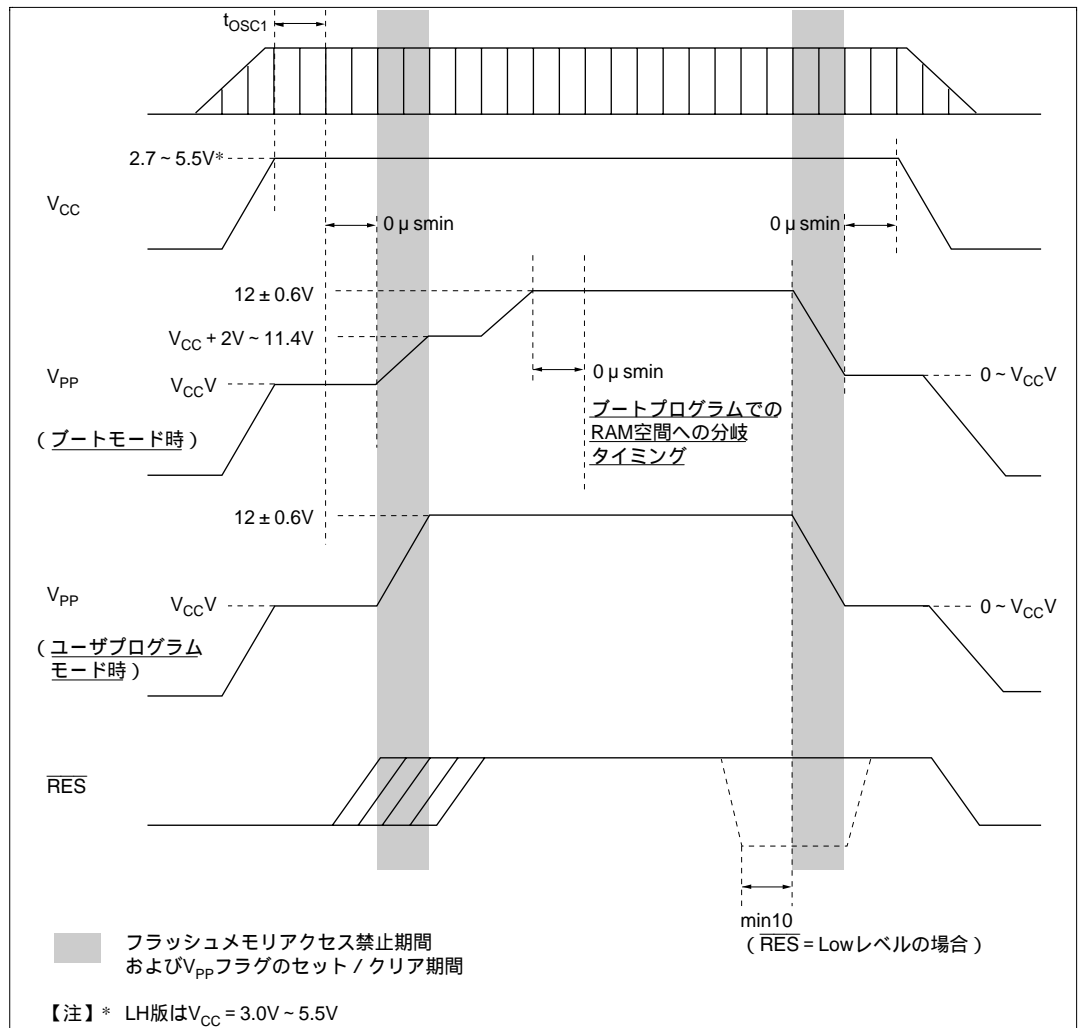
図 19.20 V_{pp} 電源投入および切断タイミング
