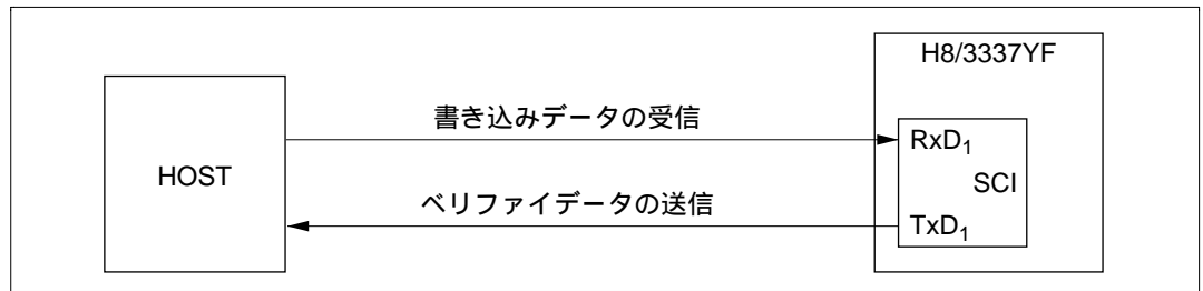
図 20.3 ブートモードシステム構成図
