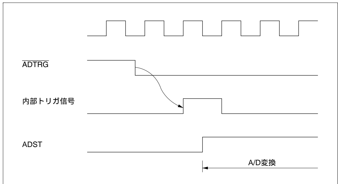
図 15.6 外部トリガ入力タイミング
