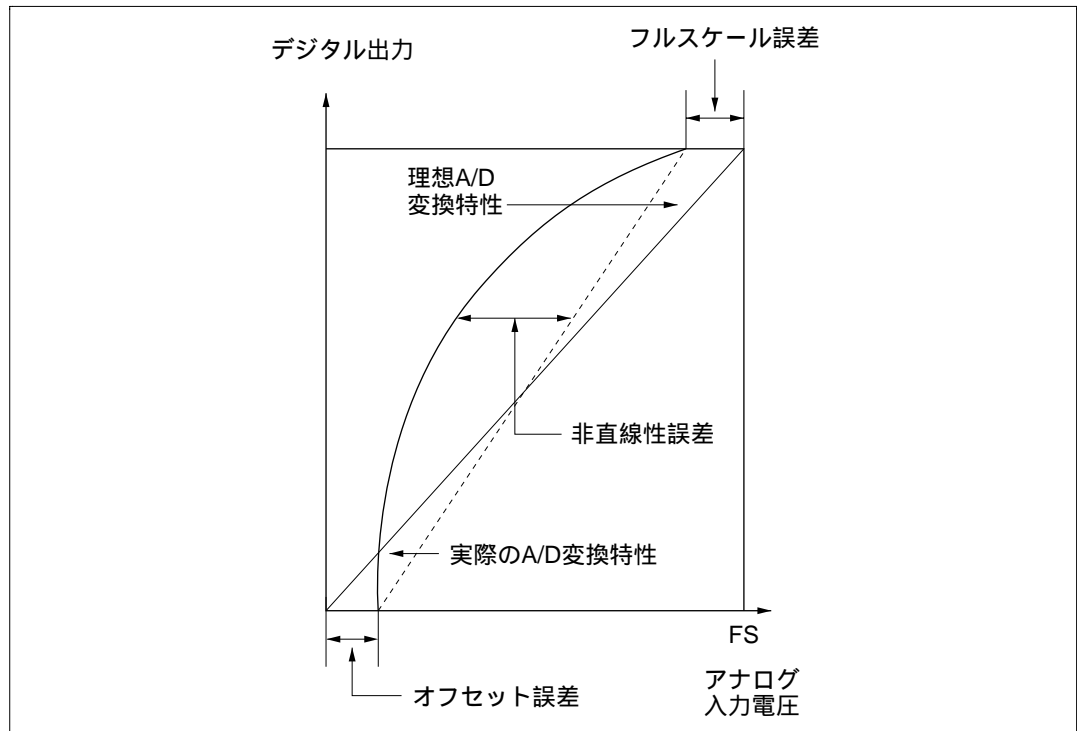
図 15.9 A/D 変換精度の定義 (2)
