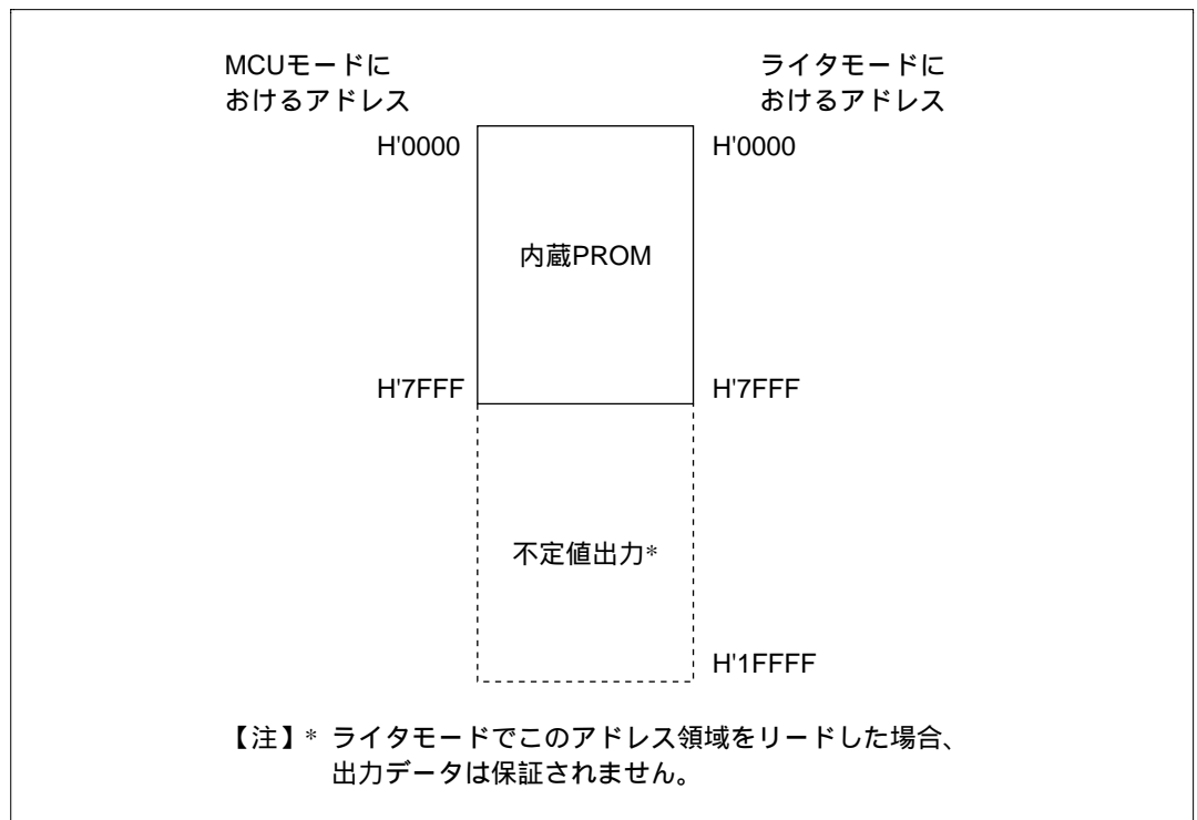
図 18.4 H8/3334Yのライタモード時のメモリマップ
