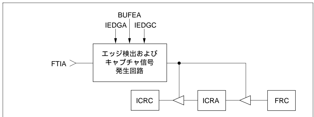
図 8.2 バッファ動作 (例)
