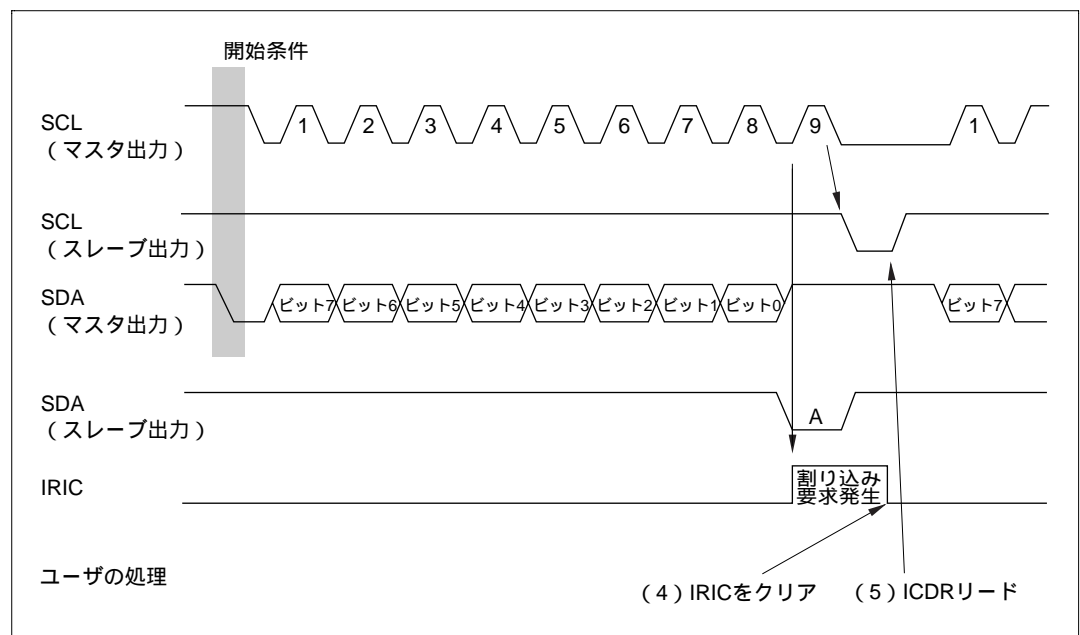
図 13.9 スレーブ受信モード動作タイミング (MLS = WAIT = ACK = ACKB = 0 のとき)
