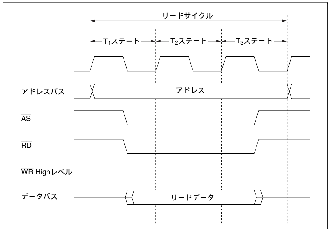
図 2.17 (a) 外部デバイスアクセスタイミング (リード時)
