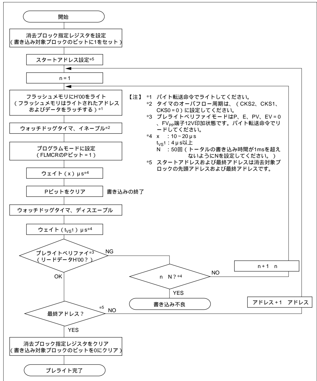
図 19.9 消去フローチャート
