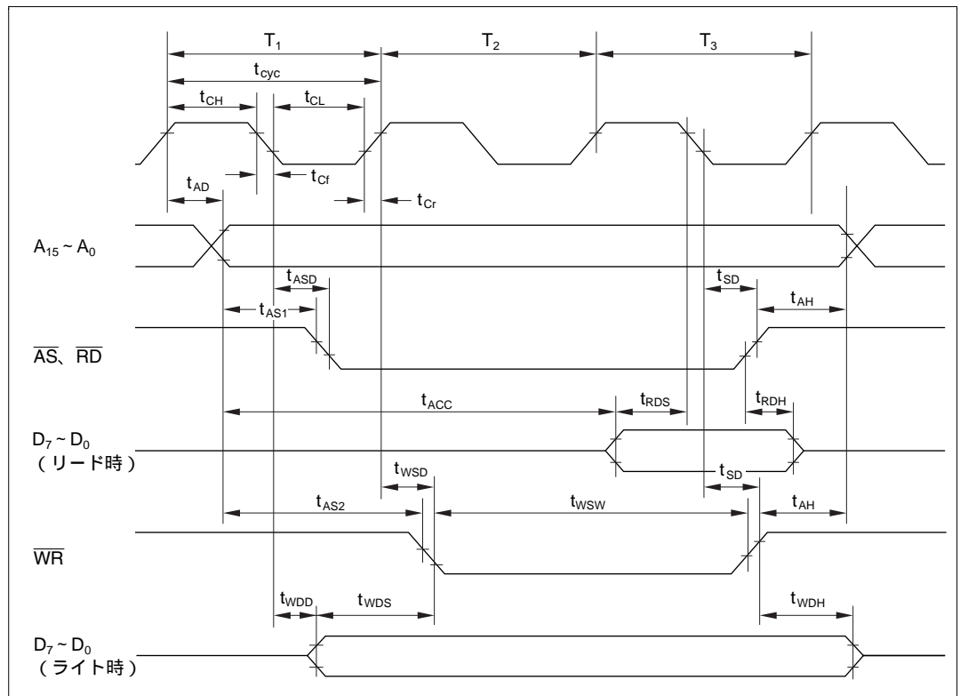
図 23.7 拡張モード時基本バスサイクル (ウェイトステートなし)
