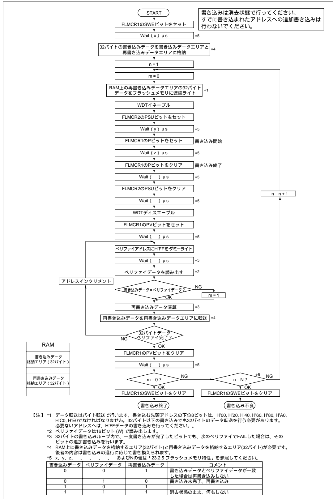
図 21.12 プログラム / プログラムベリファイフロー
