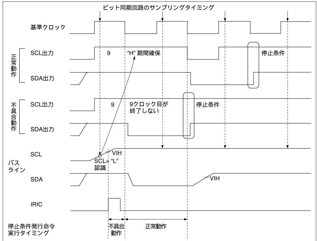
図 13.18 停止条件不具合動作タイミング
