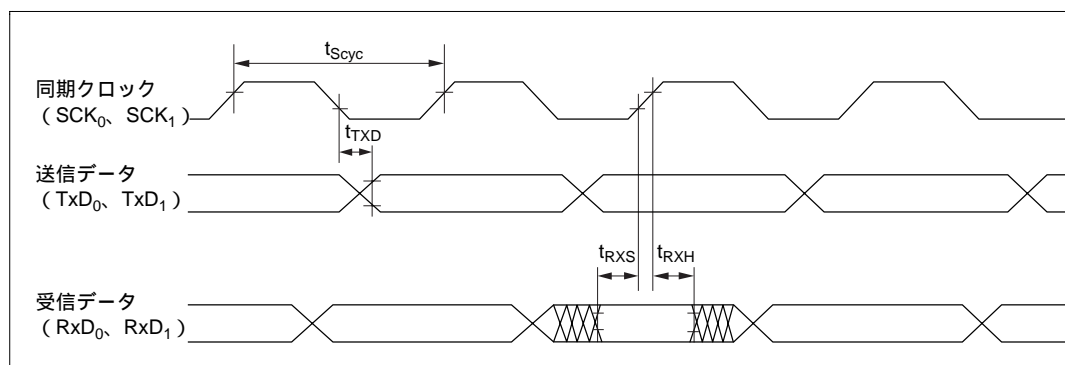
図 23.19 SCI 入出力タイミング (クロック同期モード)
