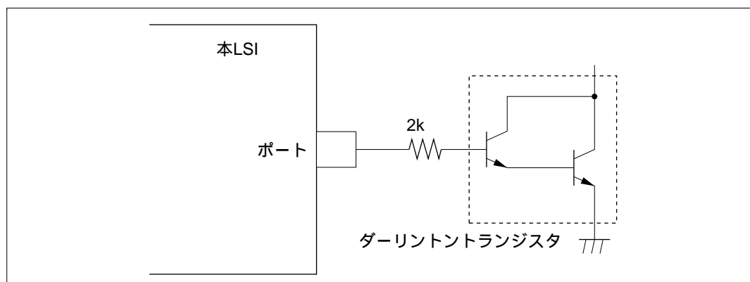
図 23.4 ダーリントントランジスタ駆動回路（5V 版の例）
