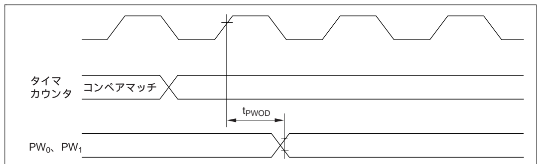
図 23.18 PWM タイマ出力タイミング
