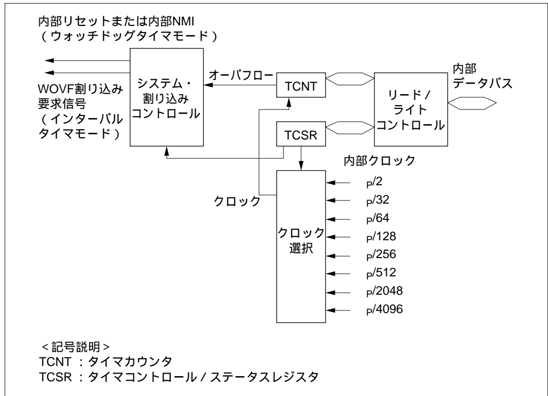
図 11.1 WDTのブロック図
