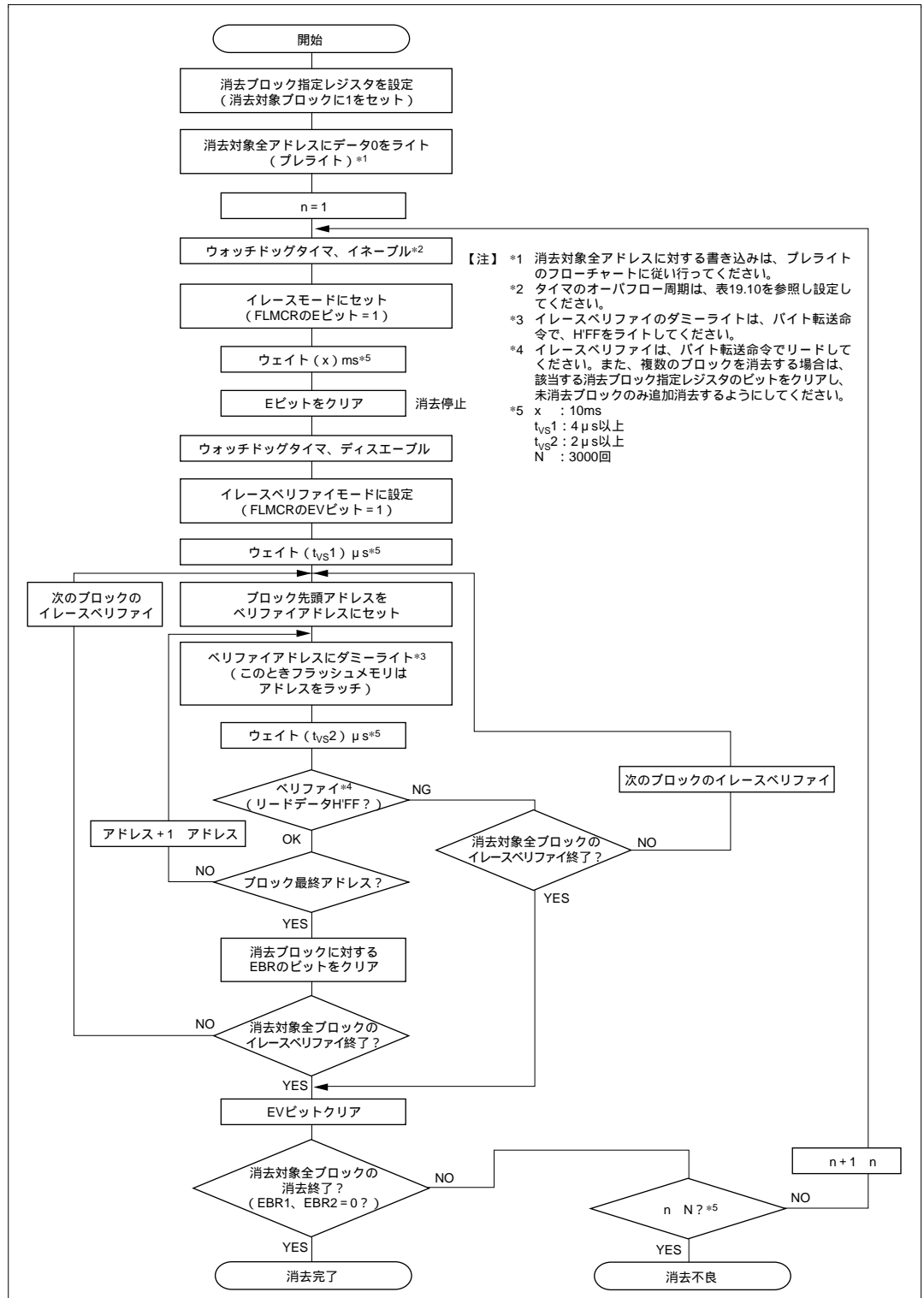
図 19.11 複数ブロック消去フローチャート
