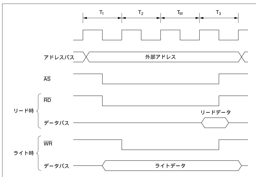
図 5.2 プログラマブルウェイトモード
