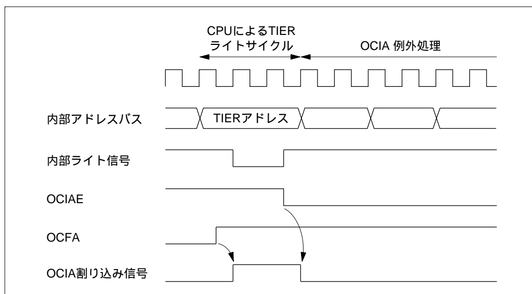
図 4.8 割り込みの発生とディスエーブルの競合
