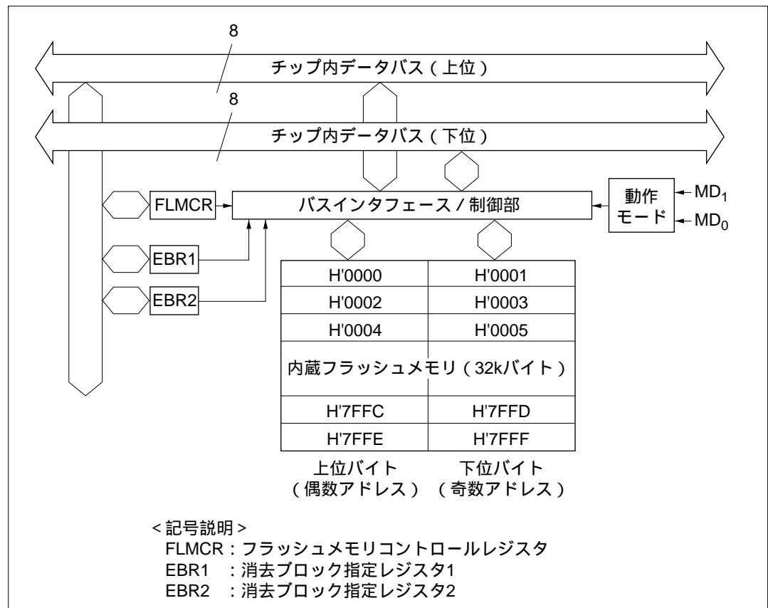
図 19.1 フラッシュメモリのブロック図
