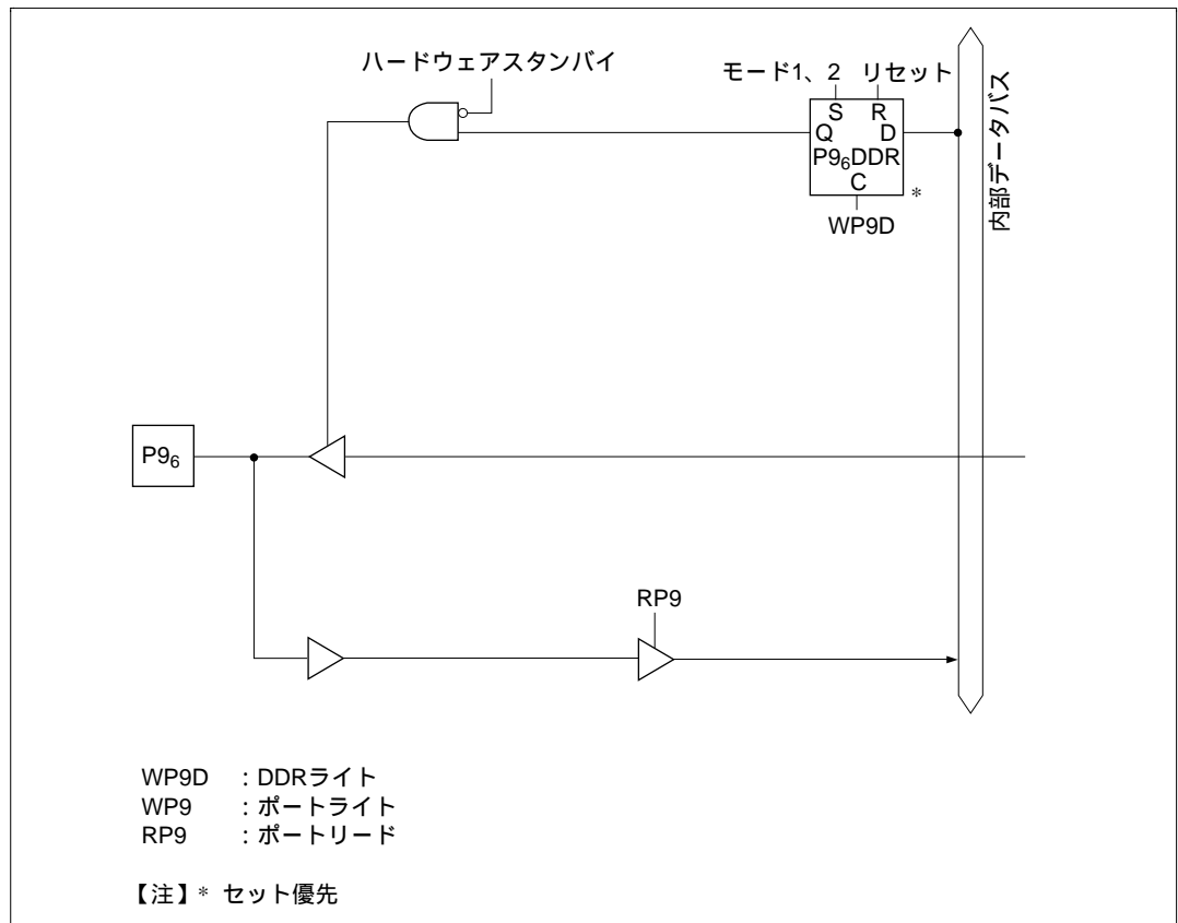
図 C.9 (e) ポート 9 ブロック図 (P9 6 端子)
