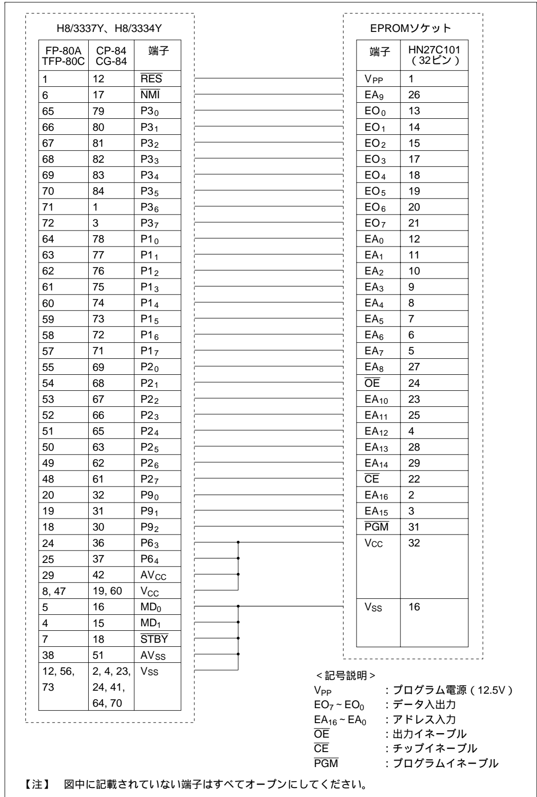
図 18.2 ソケットアダプタの端子対応図
