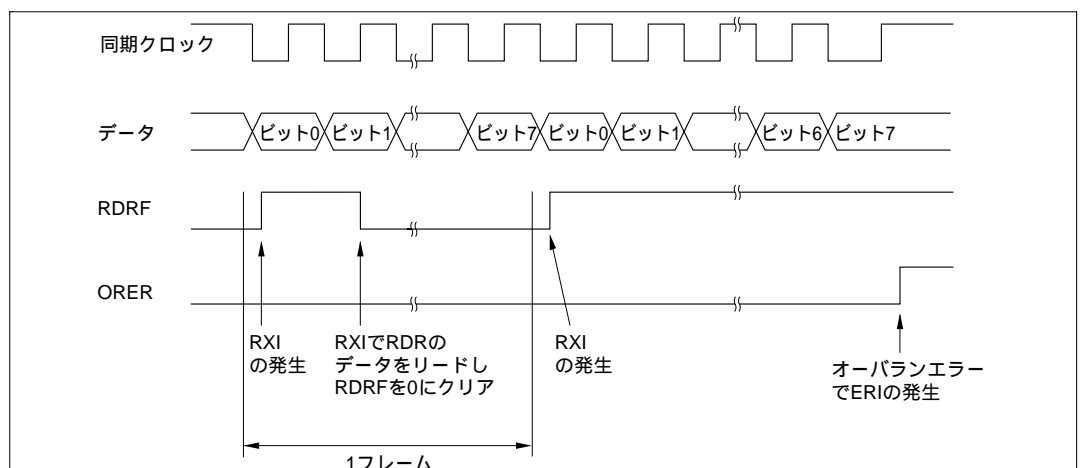
図 12.16 SCI の受信時の動作例
