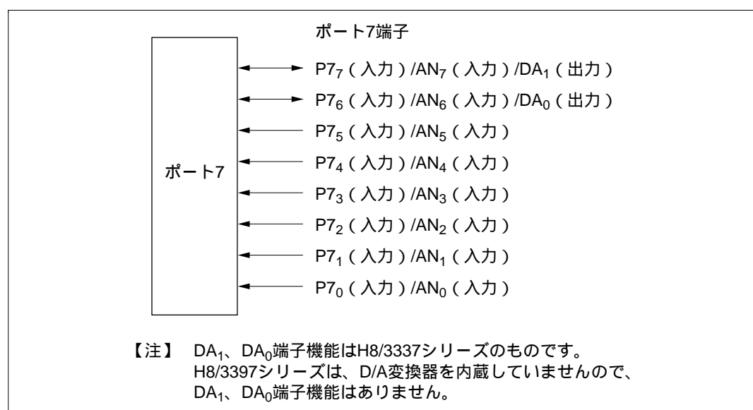
図 7.15 ポート7の端子構成
