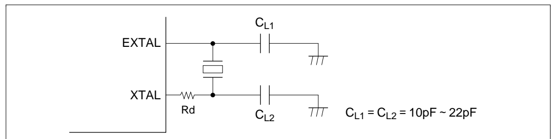
図 6.2 水晶発振子を接続する場合の接続例
