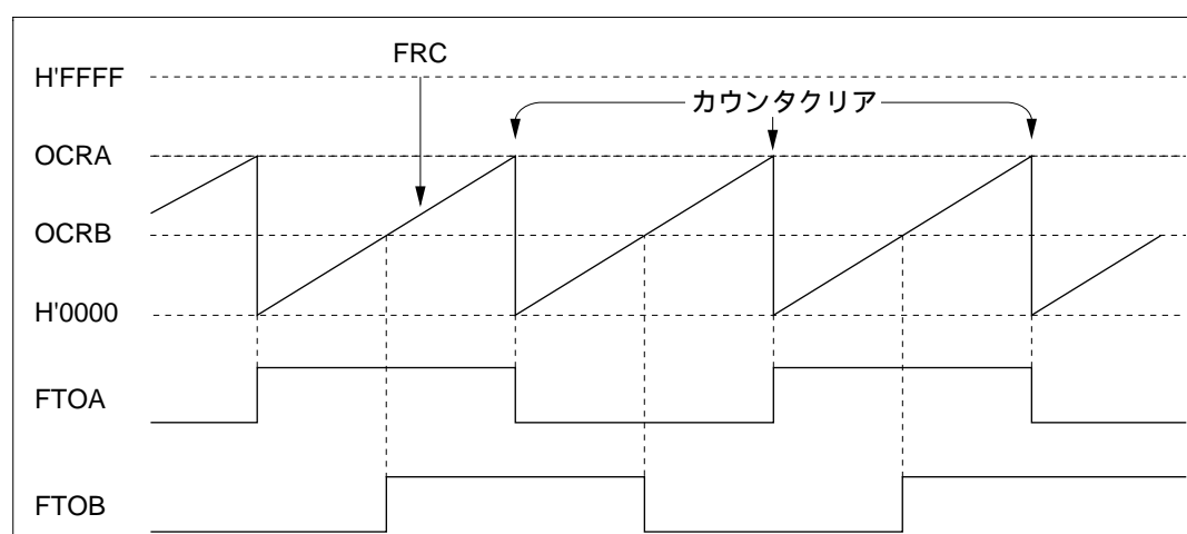
図 8.15 パルス出力例
