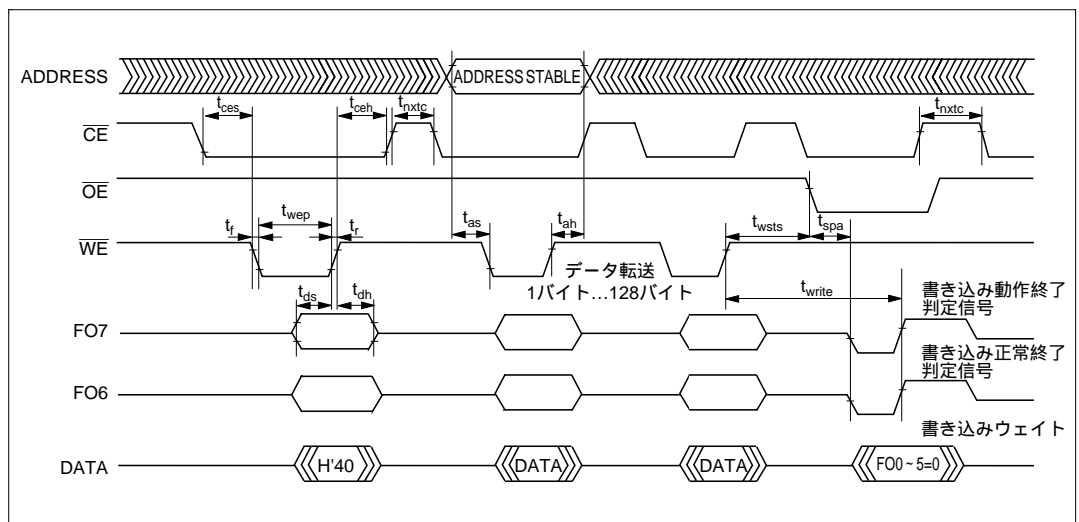
図 21.20 自動プログラムモードのタイミング波形
