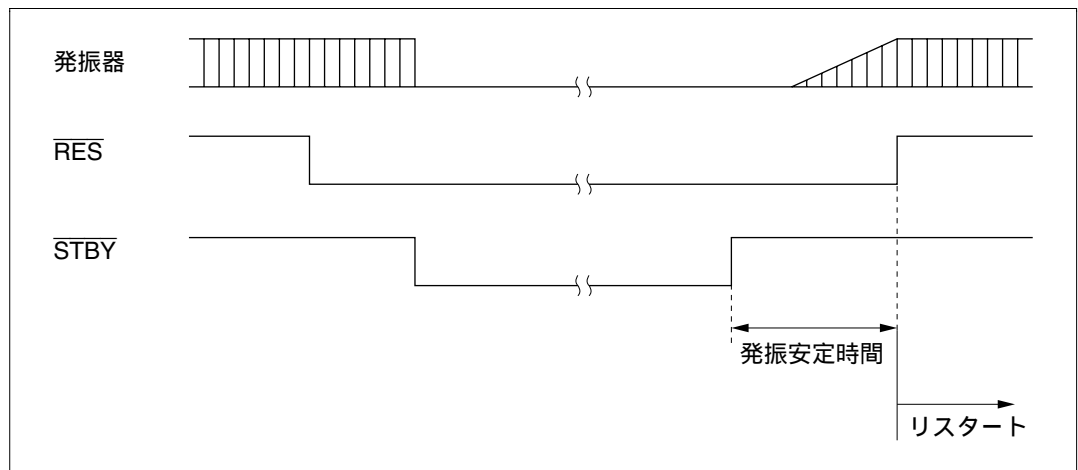
図 22.2 ハードウェアスタンバイモードのタイミング
