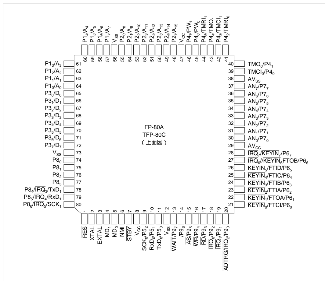
図 1.2 (b) H8/3397 シリーズのピン配置 (FP-80A、TFP-80C : 上面図)
