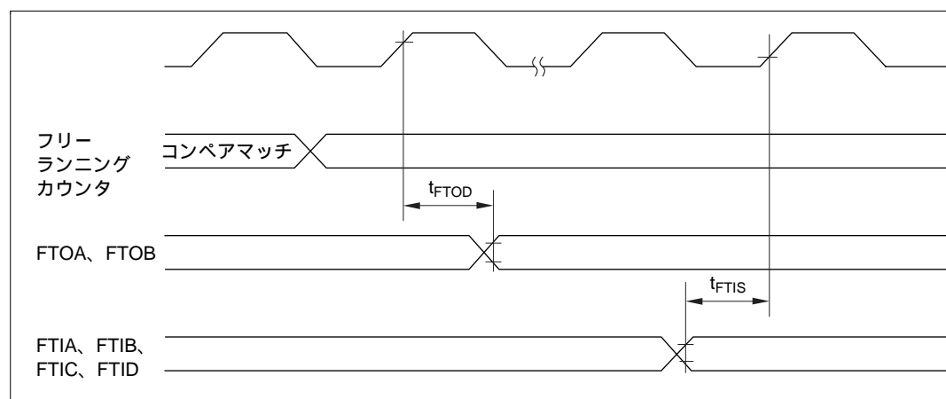
図 23.13 フリーランニングタイマ入出力タイミング
