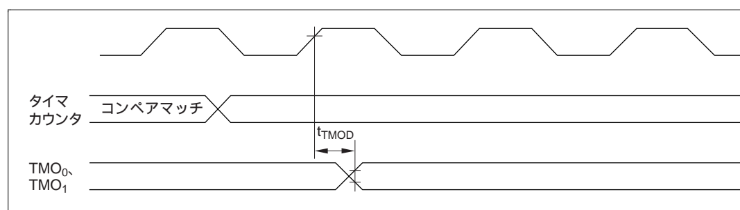
図 23.15 8ビットタイマ出力タイミング
