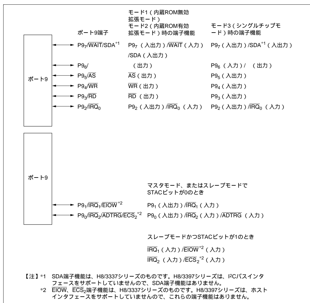
図7.17 ポート9の端子構成
