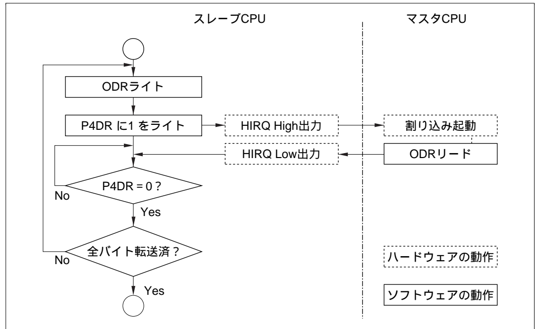
図 14.3 HIRQ の出力の利用フロー
