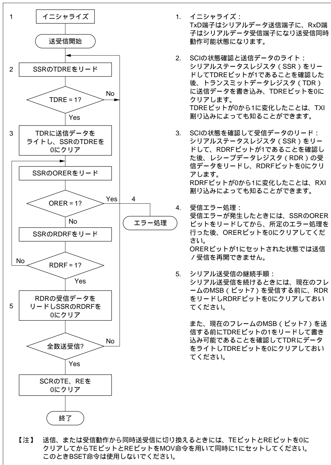
図 12.17 シリアル送受信同時動作のフローチャートの例
