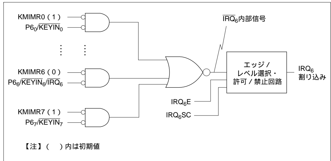
図 4.3 KMIMR と IRQ 6 割り込み
