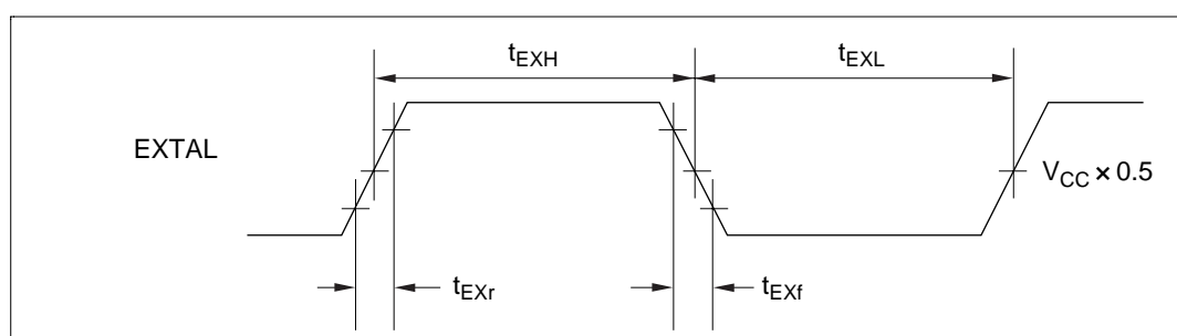
図 6.12 外部クロック入力タイミング
