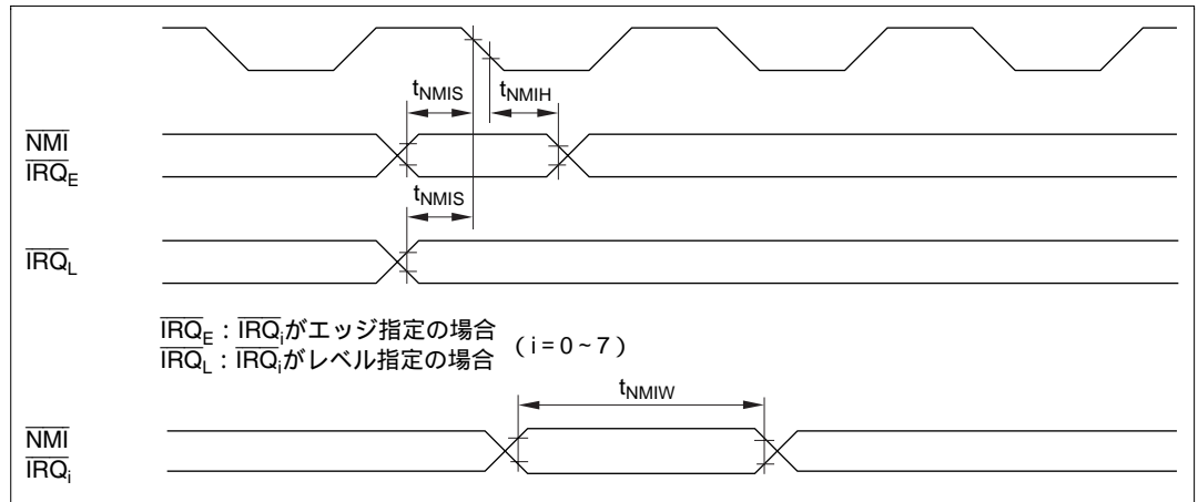
図 23.10 割り込み入力タイミング
