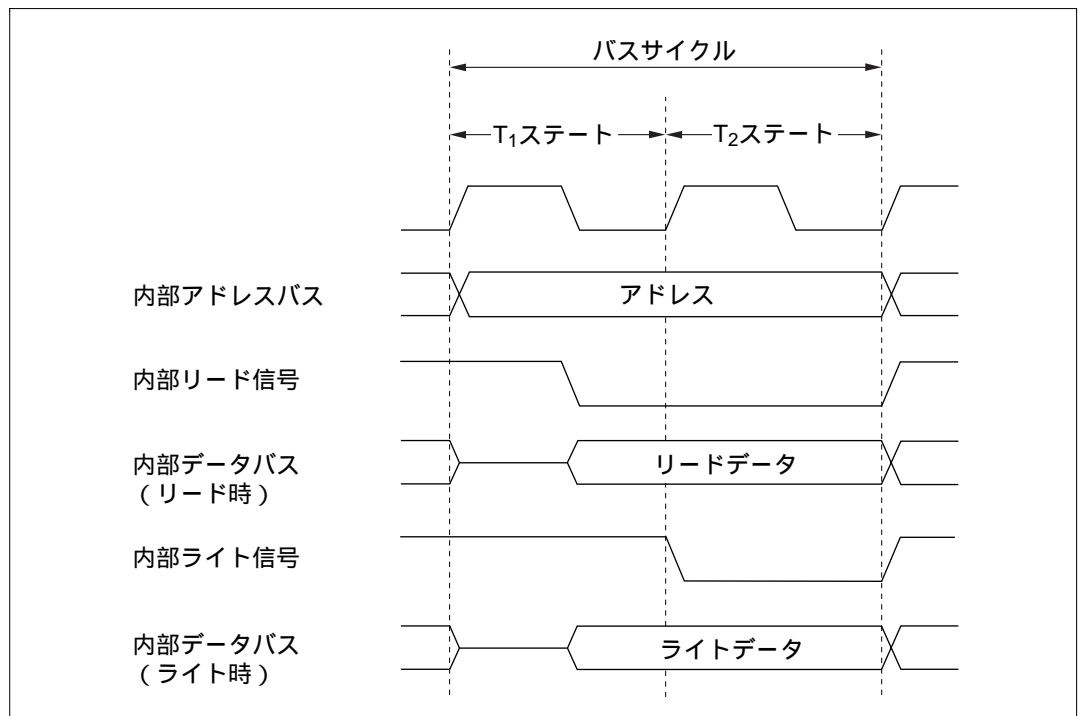
図 2.13 内蔵メモリアクセスサイクル
