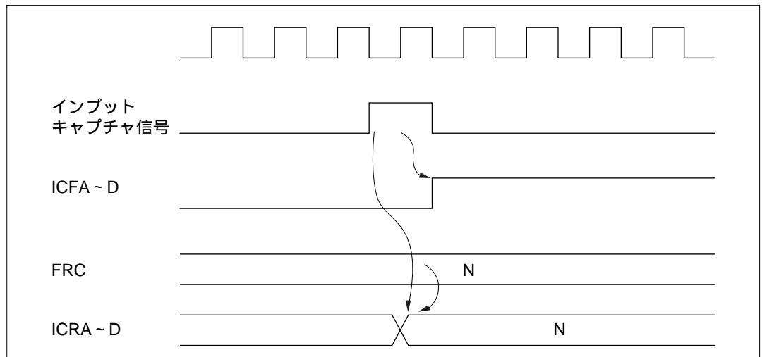
図 8.12 ICFA ~ D のセットタイミング
