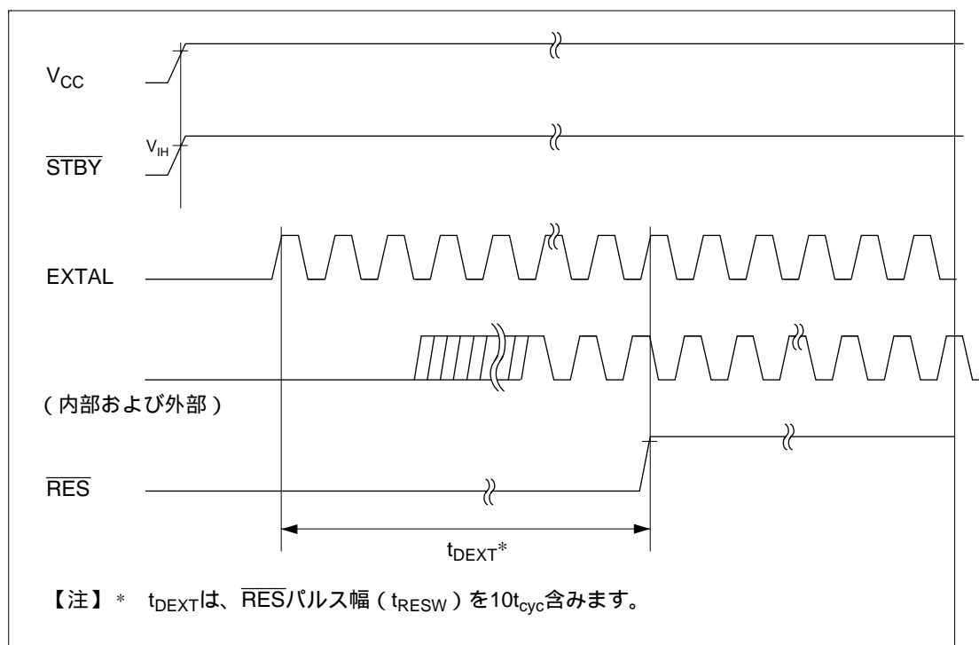
図 23.25 外部クロック出力遅延タイミング
