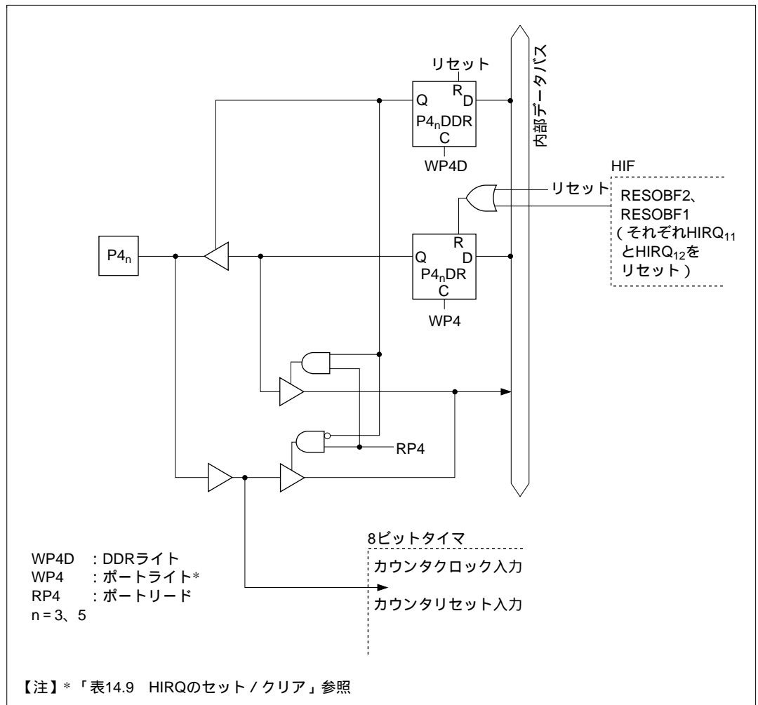
図 C.4 (c) ポート 4 ブロック図 (P4 3 、P4 5 端子)
