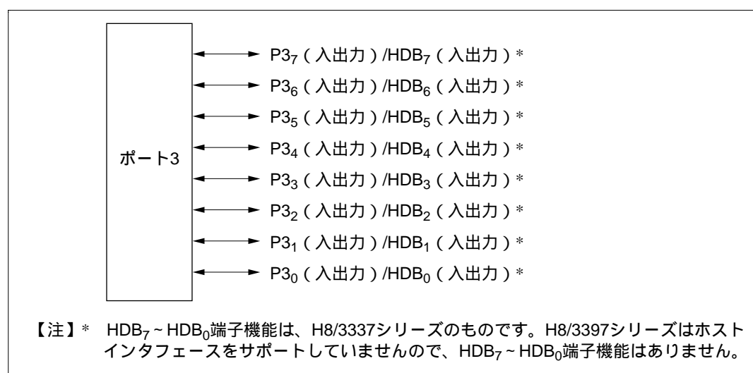
図7.11 モード3の端子機能(ポート3)
