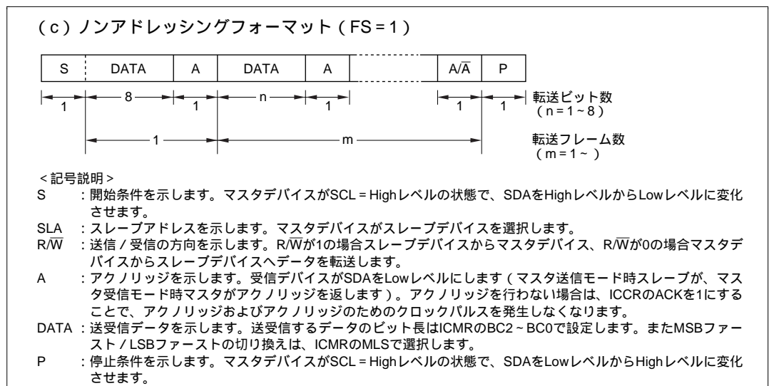
図 13.4 I 2 C バスデータフォーマット (ノンアドレッシングフォーマット)
