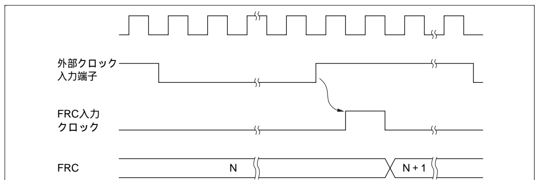
図 8.5 外部クロック動作時のカウントタイミング
