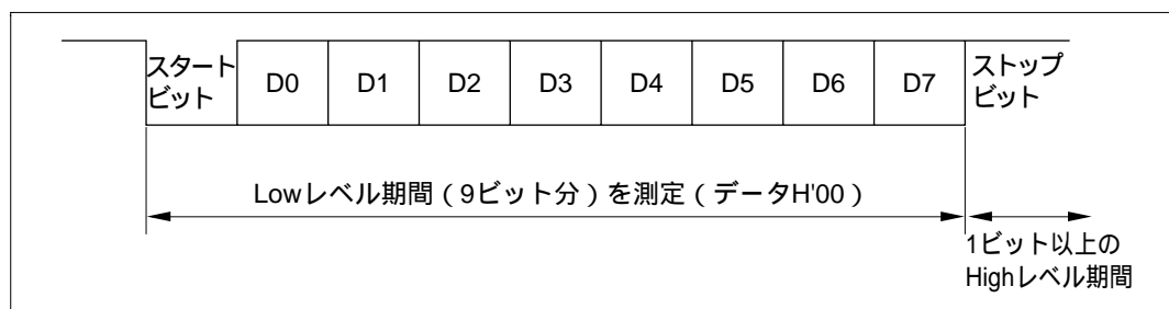
図 20.5 ホスト送信データの Low レベル期間の測定
