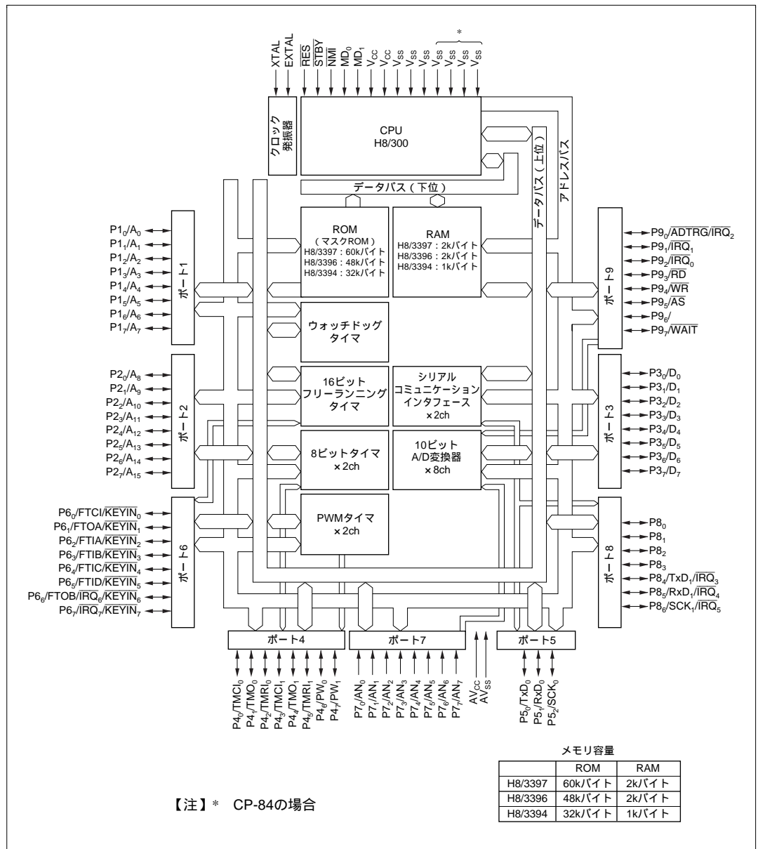
図 1.1 (b) H8/3397 シリーズの内部ブロック図
