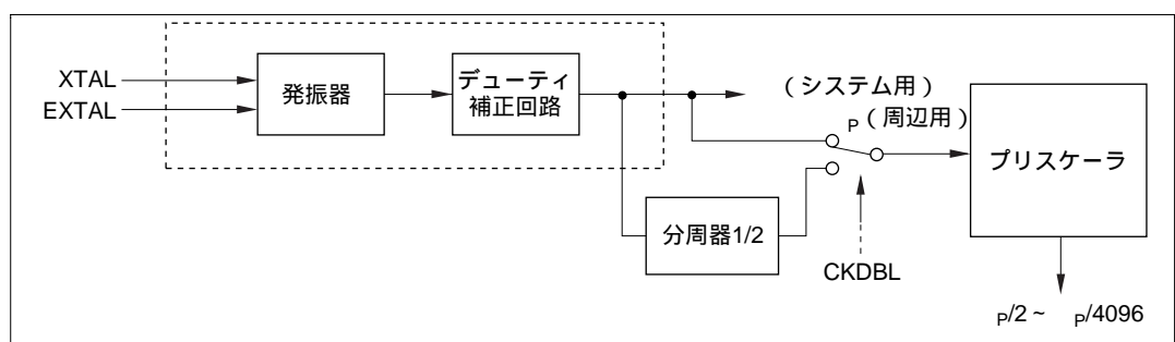
図 6.1 クロック発振器のブロック図
