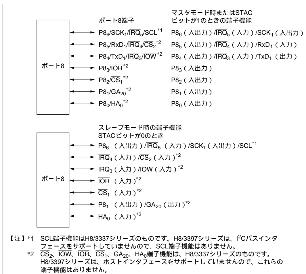
図 7.16 ポート 8 の端子構成
