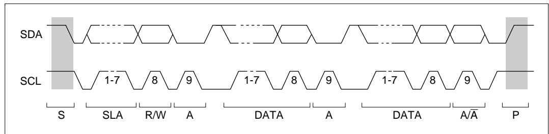
図 13.5 I 2 C バスタイミング
