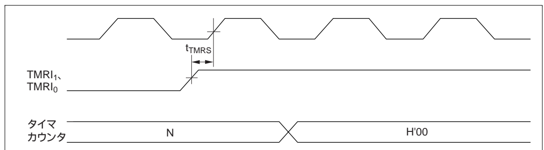
図 23.17 8ビットタイマリセット入力タイミング
