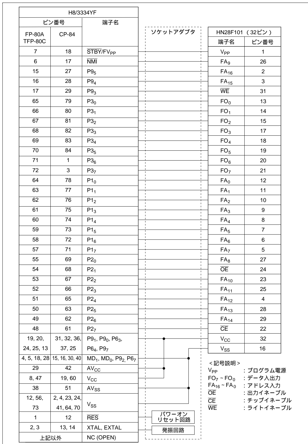
図 19.14 ソケットアダプタの端子対応図
