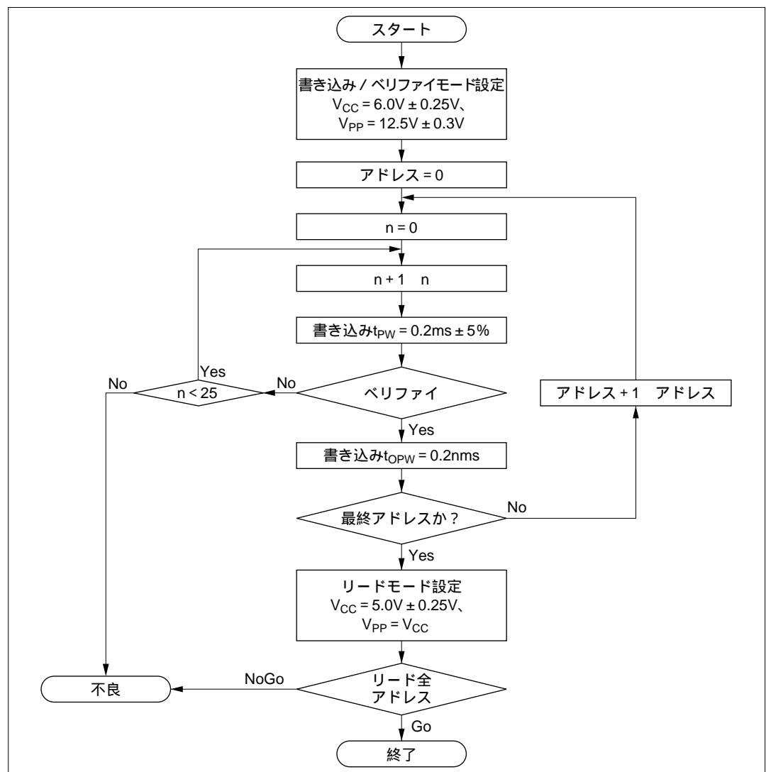
図 18.5 高速プログラミングフローチャート
