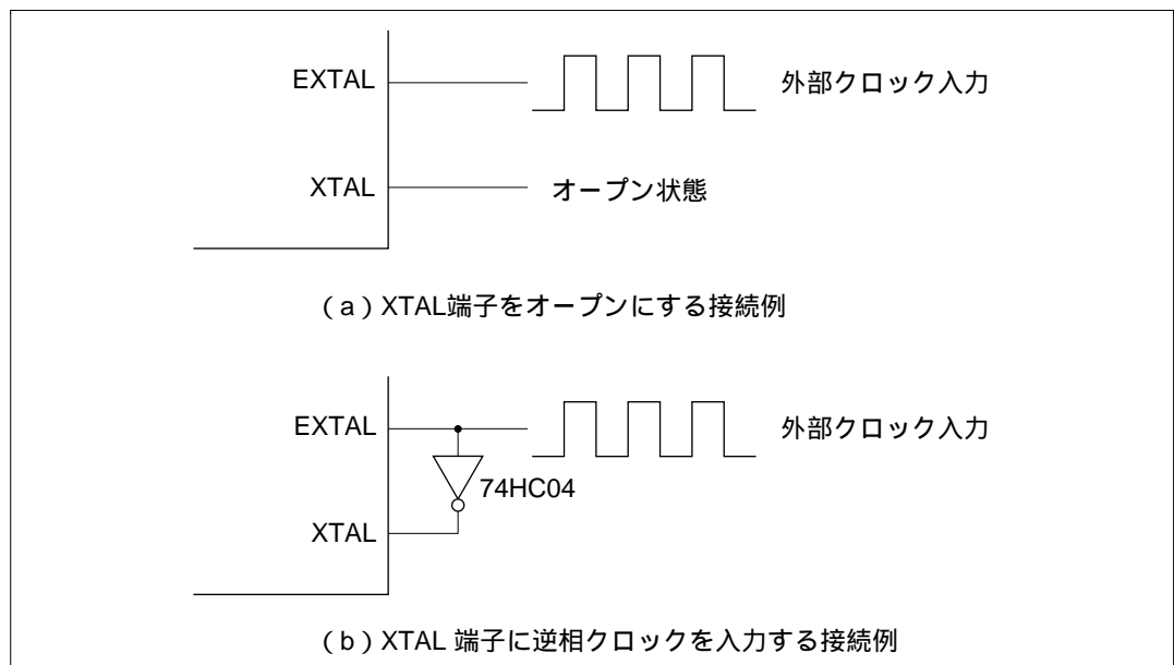
図 6.11 外部クロックを入力する場合の接続例
