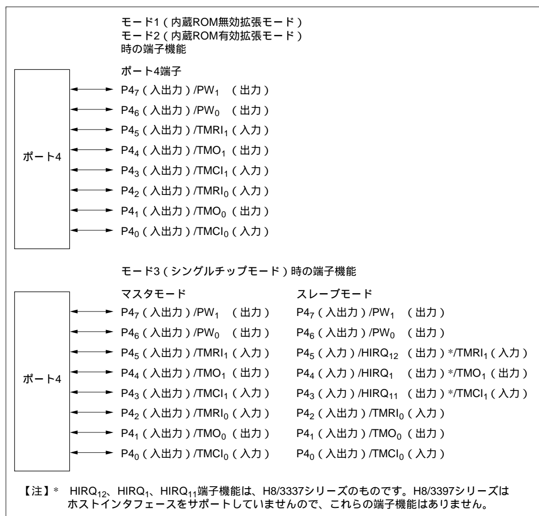
図7.12 ポート4の端子構成
