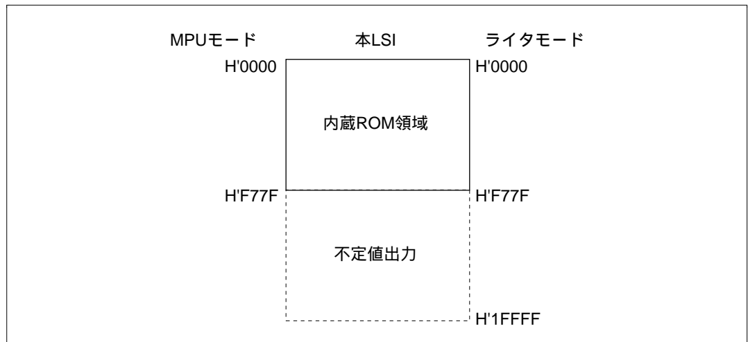
図 21.15 ライタモード時のメモリマップ
