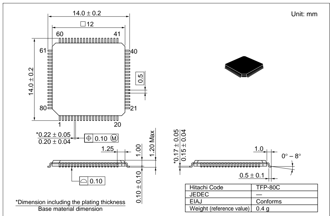
図 I.2 外形寸法図 (TFP-80C)
