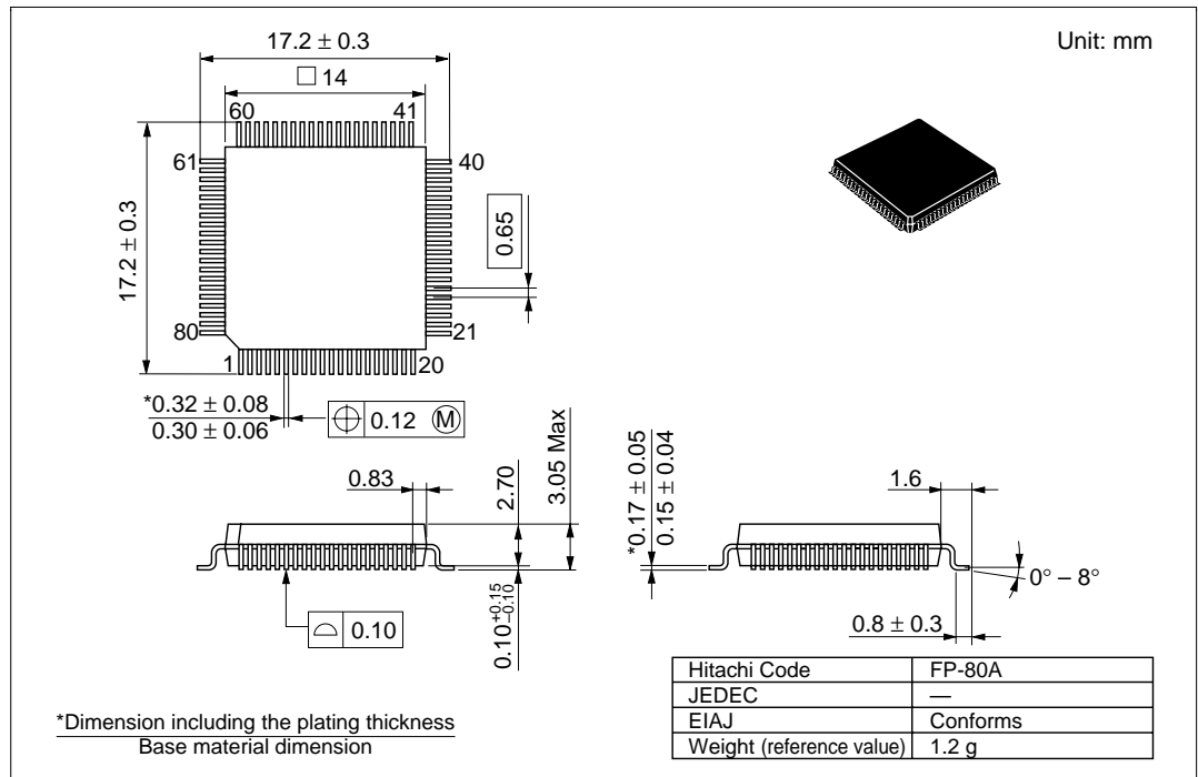
図 I.1 外形寸法図 (FP-80A)
