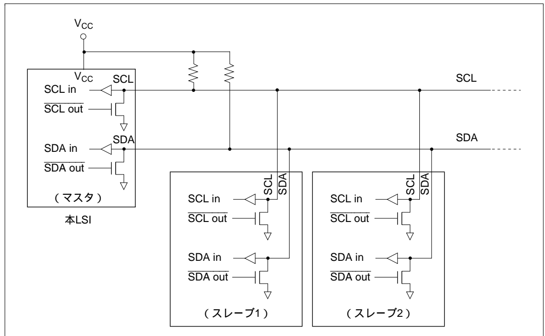
図 13.1 I 2 C バスインタフェース接続例 (本 LSI がマスタの場合)
