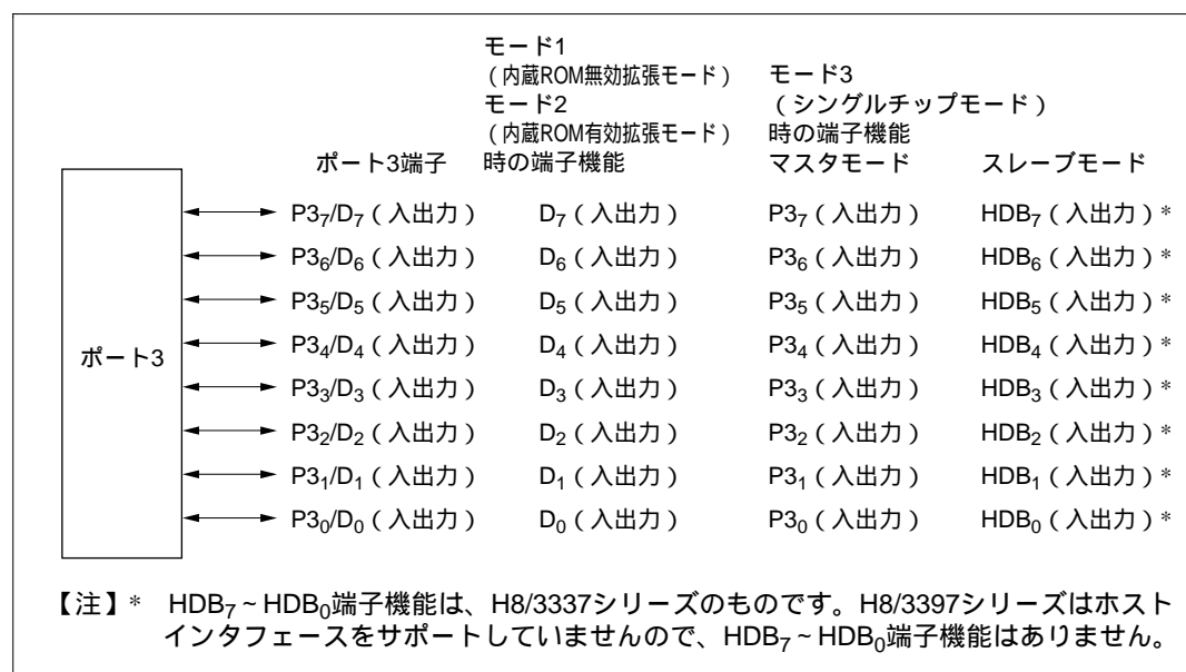
図7.9 ポート3の端子構成
