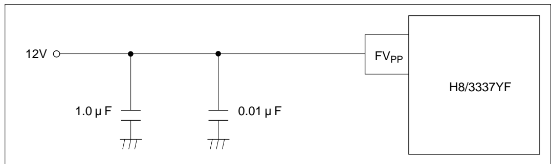
図 20.21 V_{PP} 電源回路設計例
