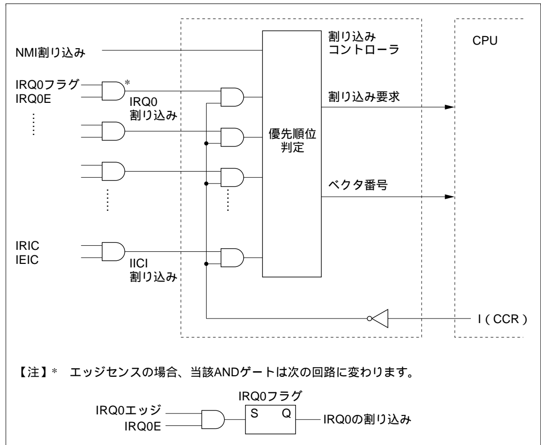
図4.4 割り込みコントローラのブロック図
