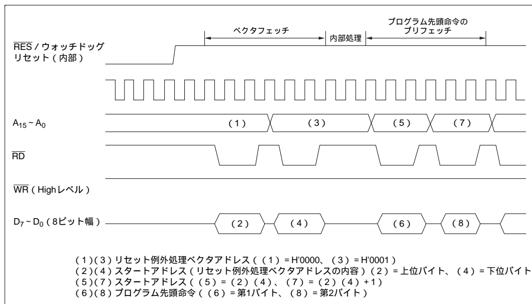
図 4.2 リセットシーケンス (モード1)
