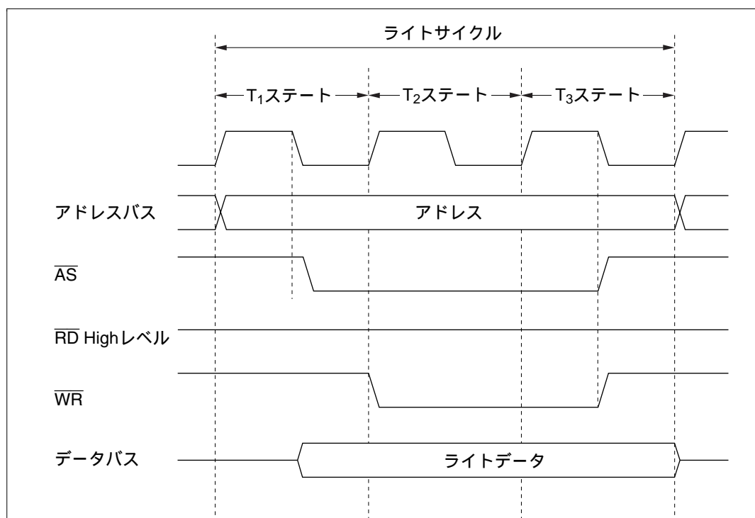
図 2.17 (b) 外部デバイスアクセスタイミング (ライト時)
