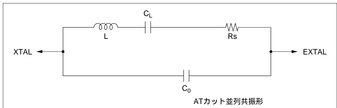
図 6.9 水晶発振子の等価回路
