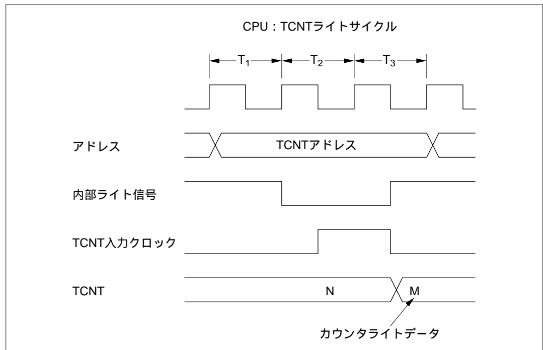
図 11.6 TCNT のライトとカウントアップの競合
