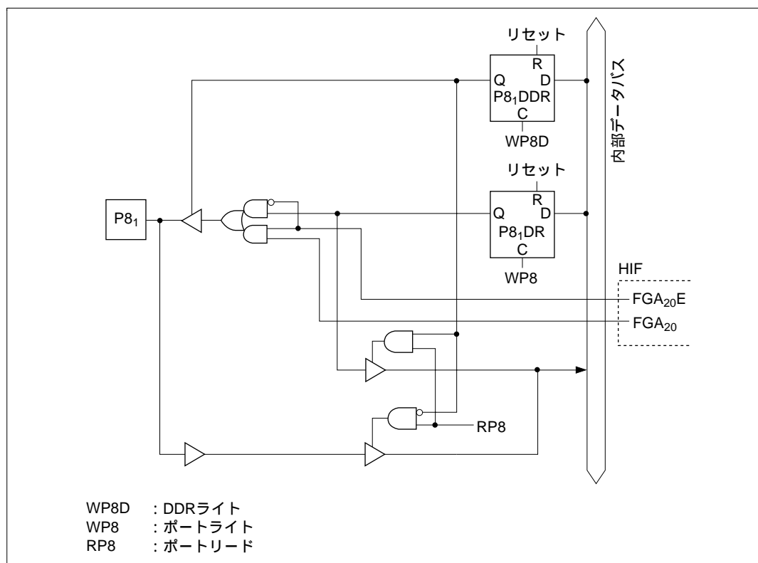
図 C.8 (b) ポート 8 ブロック図 (P8 1 端子)
