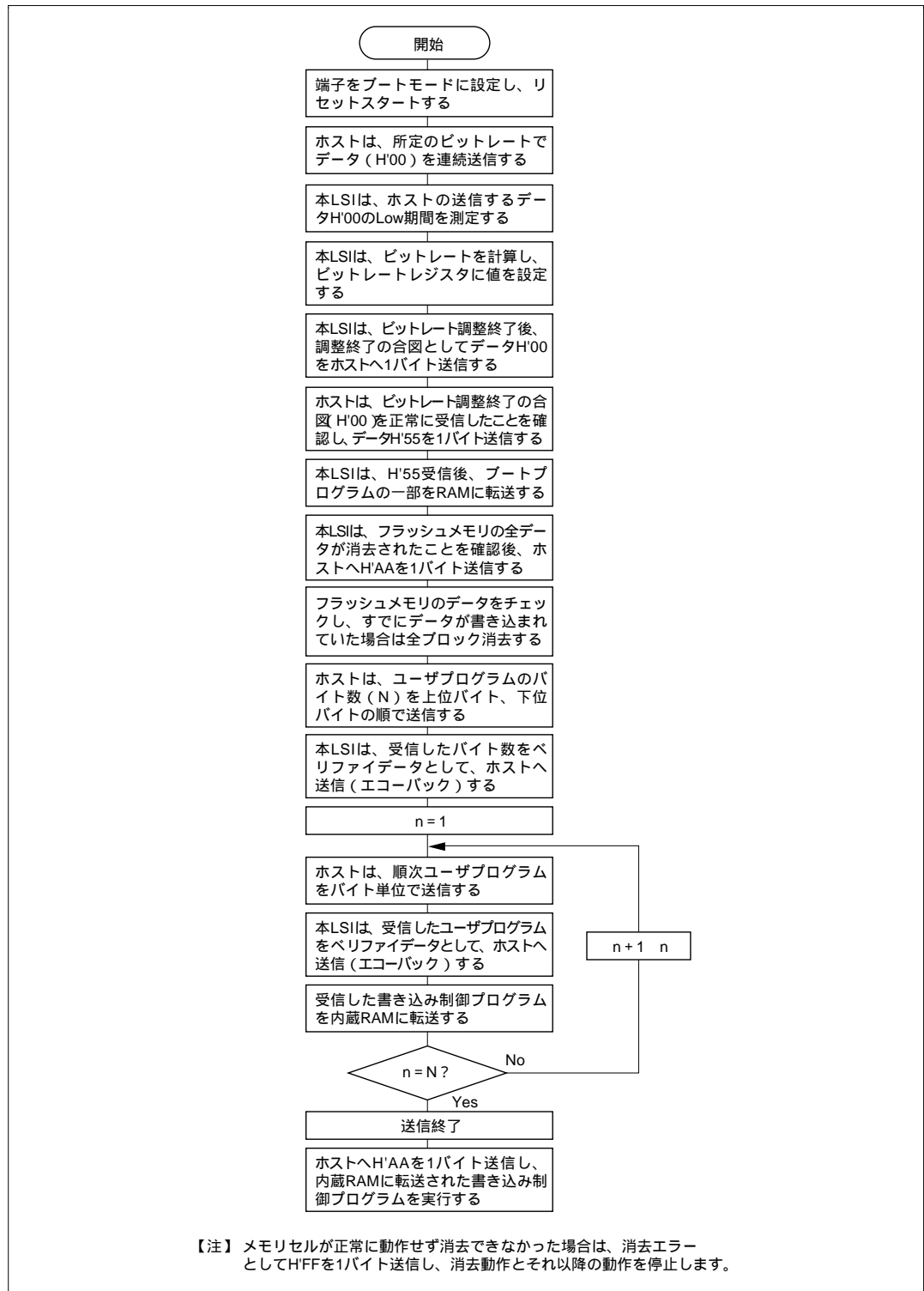
図 21.7 ブートモード実行手順
