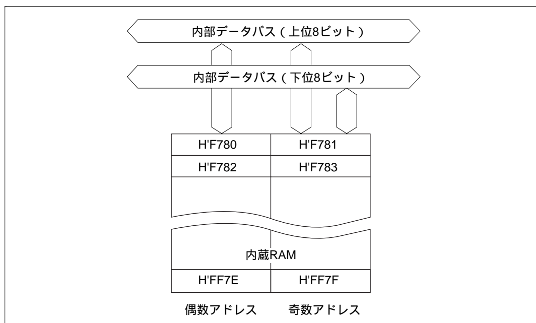
図 17.1 RAM のブロック図 (H8/3337Y の場合)
