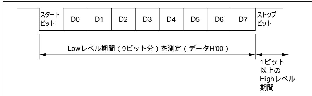
図 19.5 ホスト送信データの Low レベル期間の測定
