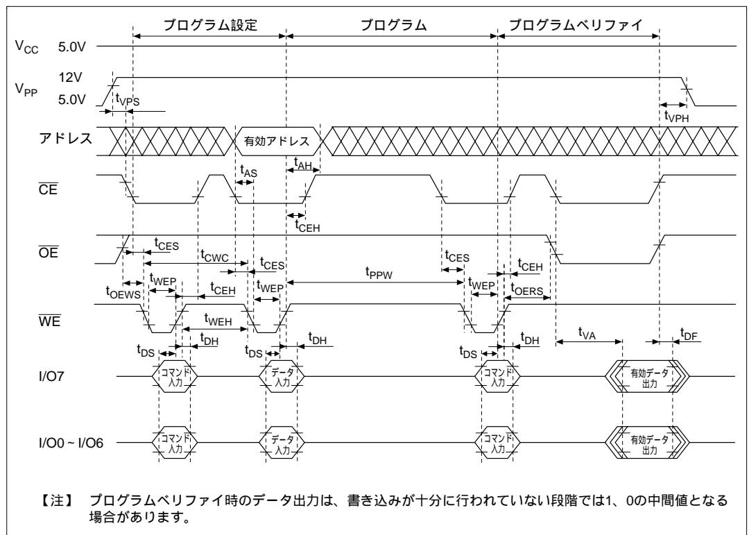
図 20.18 高速高信頼度プログラムタイミング
