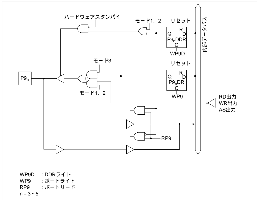
図 C.9 (d) ポート9 ブロック図 ( P9 3 、 P9 4 、 P9 5 端子 )
