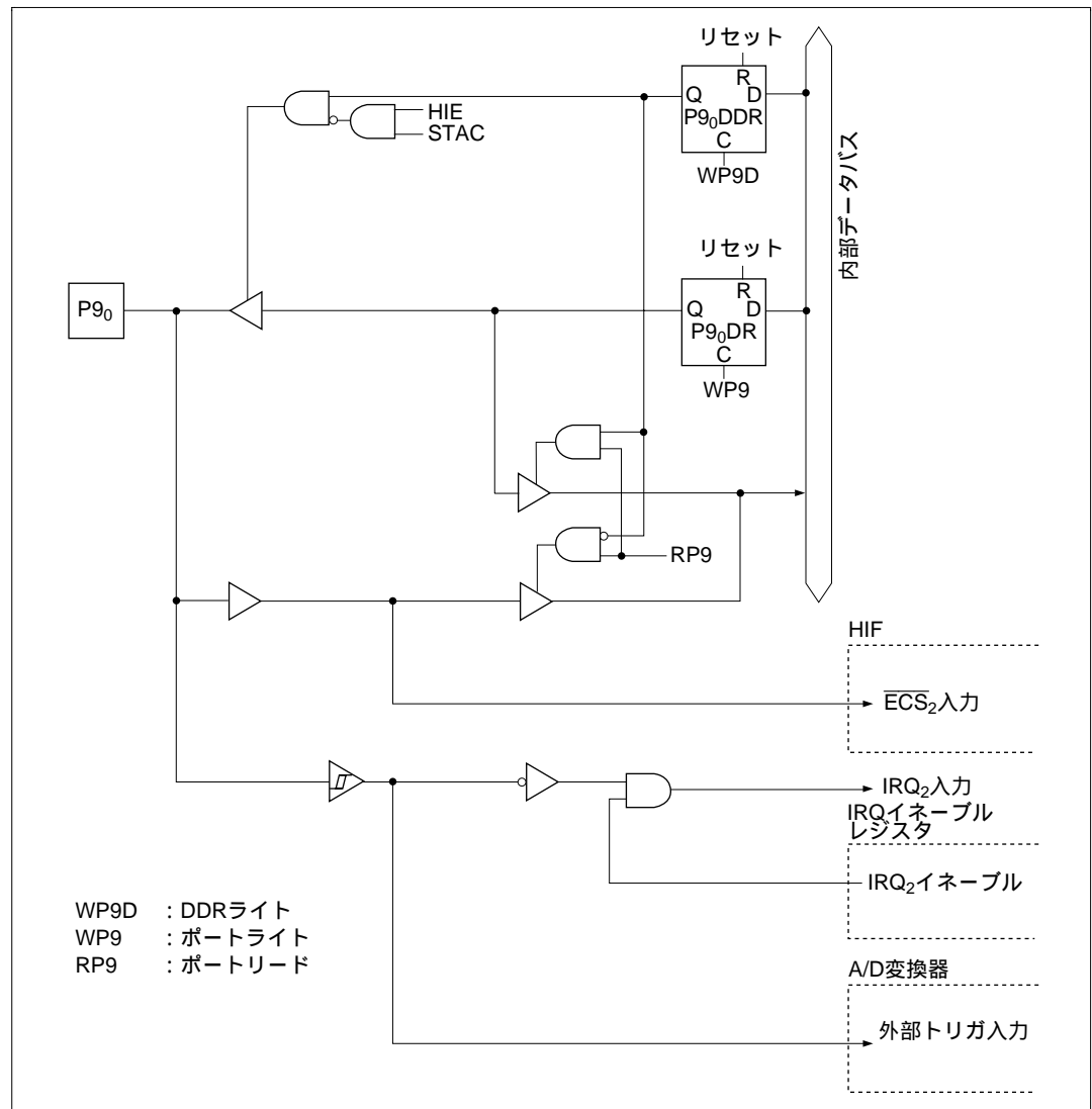
図 C.9 (a) ポート9 ブロック図 (P9 0 端子)
