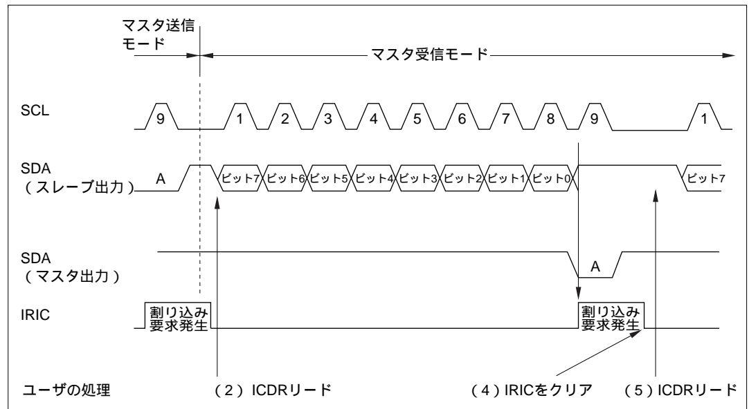
図 13.7 マスタ受信モード動作タイミング (MLS = WAIT = ACK = ACKB = 0 のとき)
