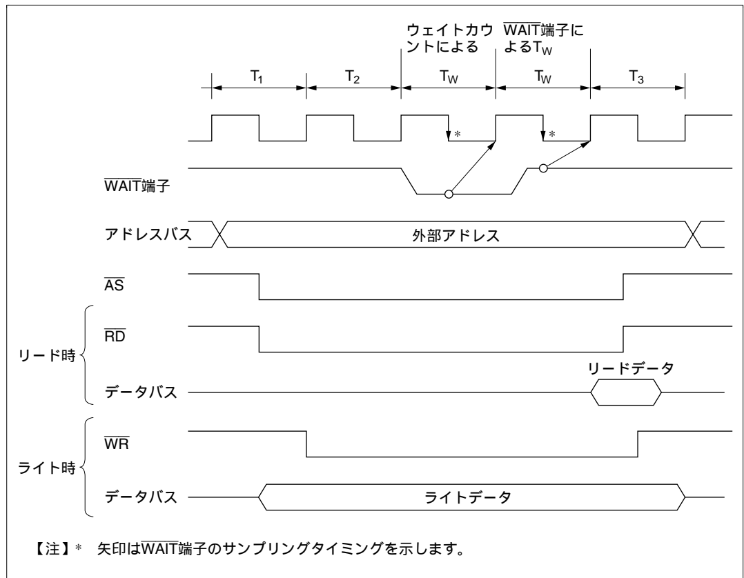
図 5.3 端子ウェイトモード
