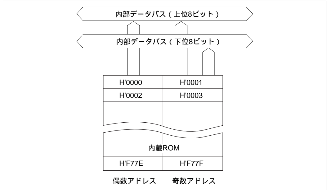
図18.1 ROMのブロック図 (H8/3337Y シングルチップモードの場合)
