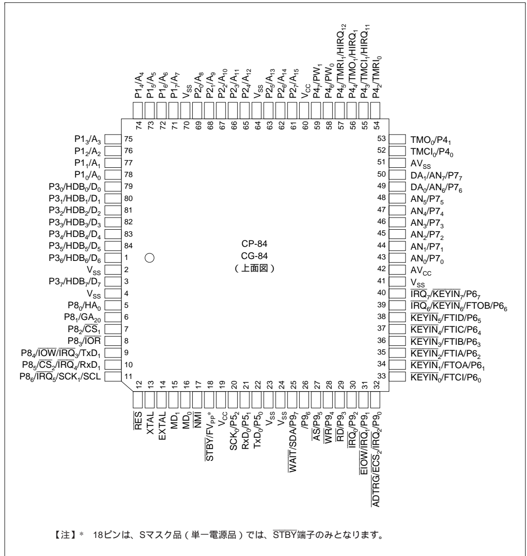
図 1.3 (a) H8/3337 シリーズのピン配置 (CP-84、CG-84 : 上面図)
