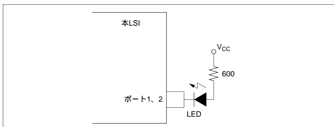
図 23.5 LED 駆動回路（5V 版の例）
