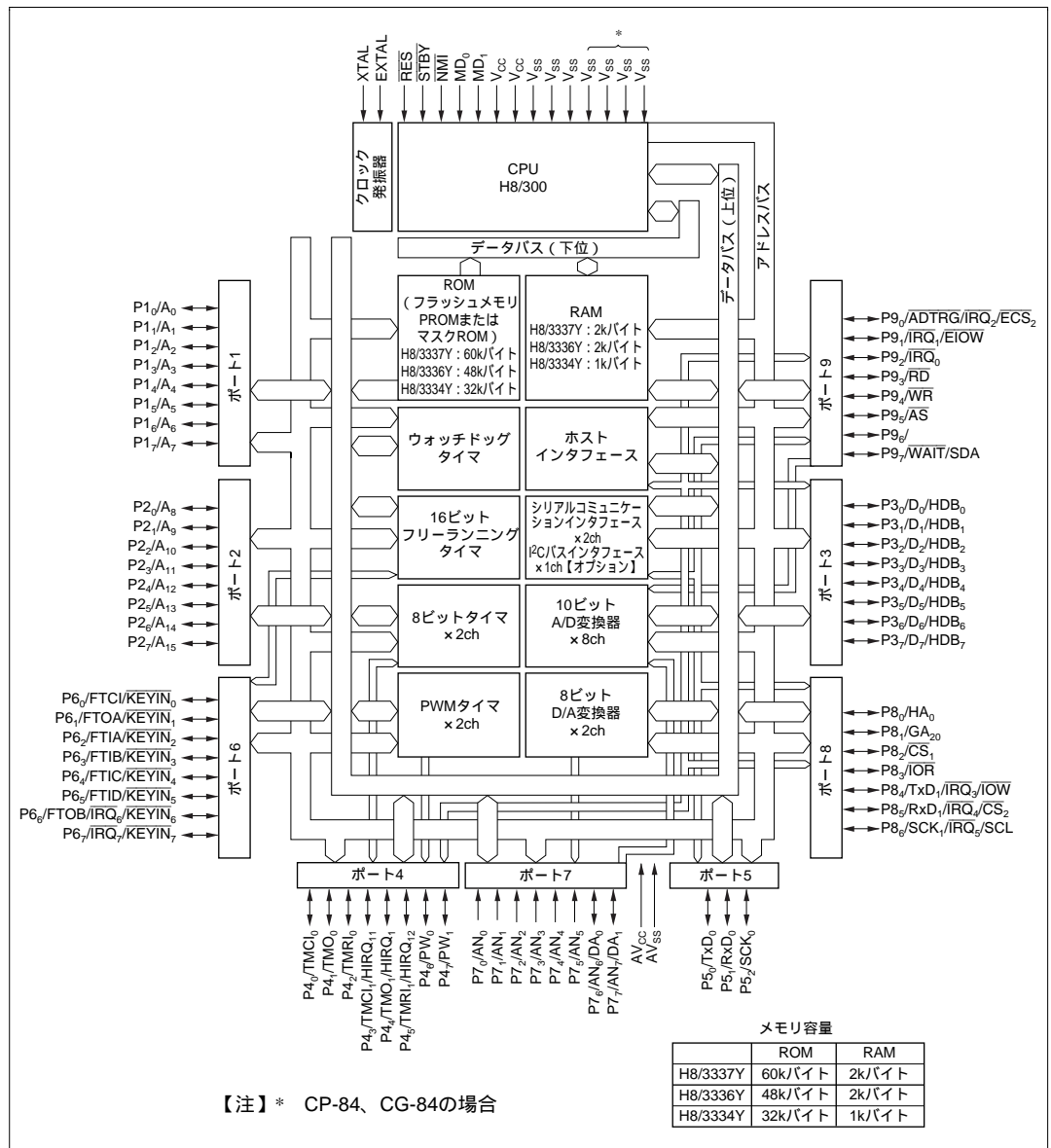
図 1.1 (a) H8/3337シリーズの内部ブロック図
