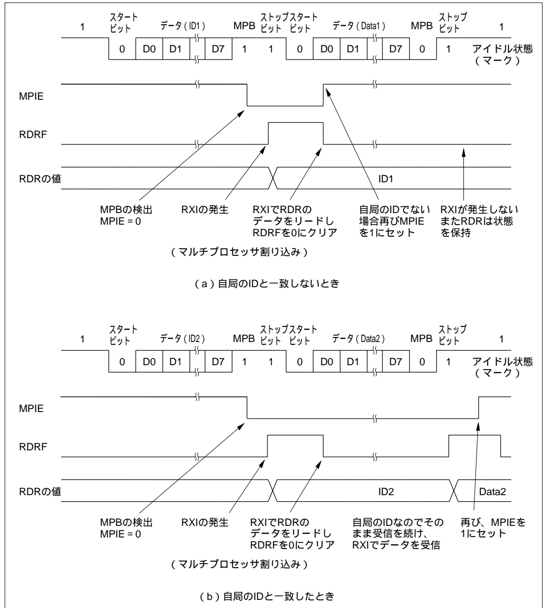
図 12.11 SCI の受信時の動作例 （8 ビットデータ / マルチプロセッサビットあり / 1 ストップビットの例）
