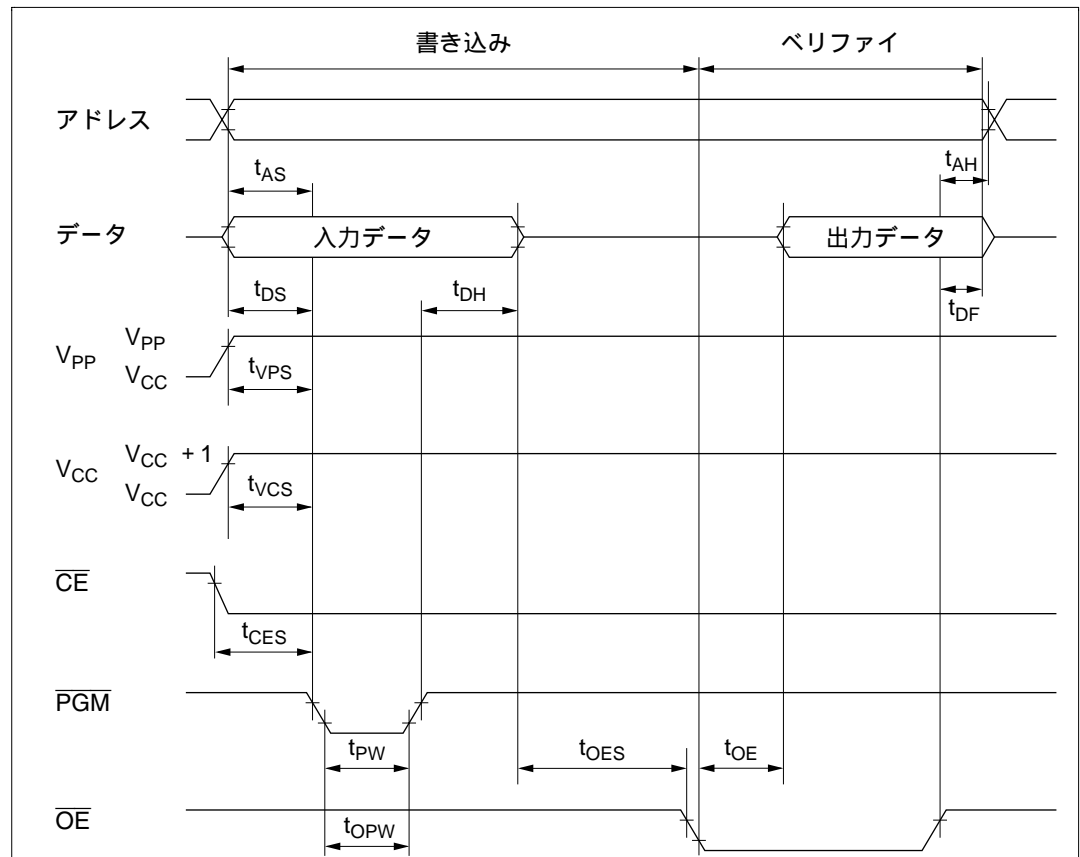
図 18.6 PROM 書き込み / ベリファイタイミング
