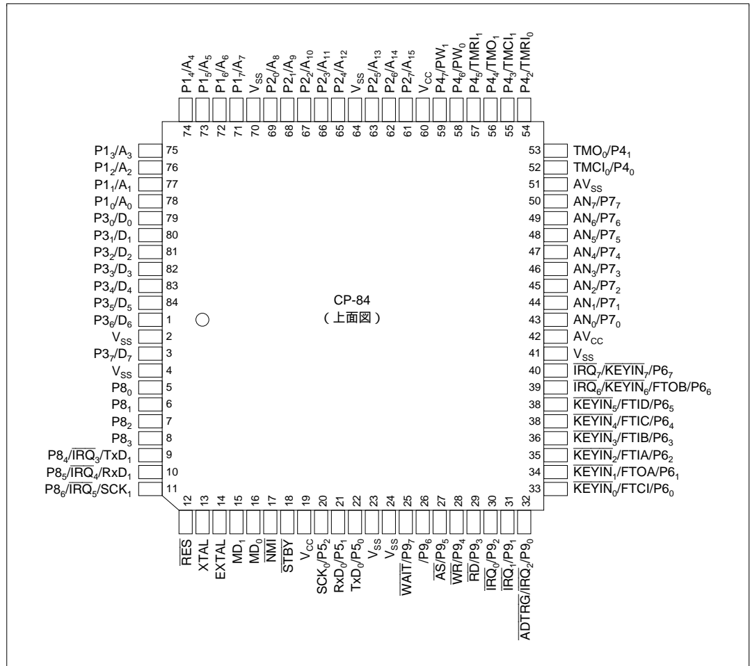
図 1.3 (b) H8/3397 シリーズのピン配置 (CP-84 : 上面図)
