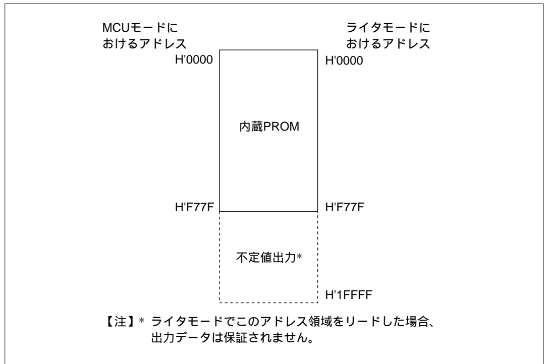
図 18.3 H8/3337Yのライタモード時のメモリマップ
