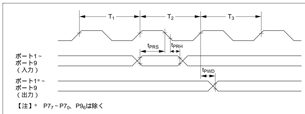
図 23.21 I/O ポート入出力タイミング
