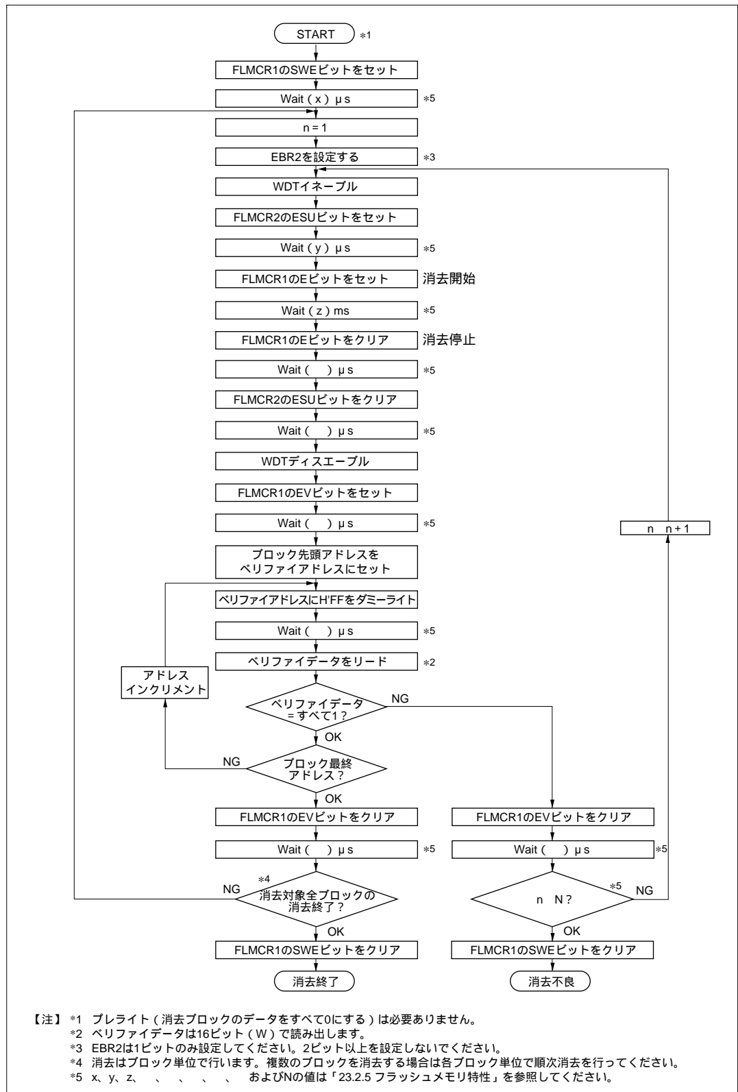
図 21.13 イレース/イレースペリファイフロー (単一ブロック消去)
