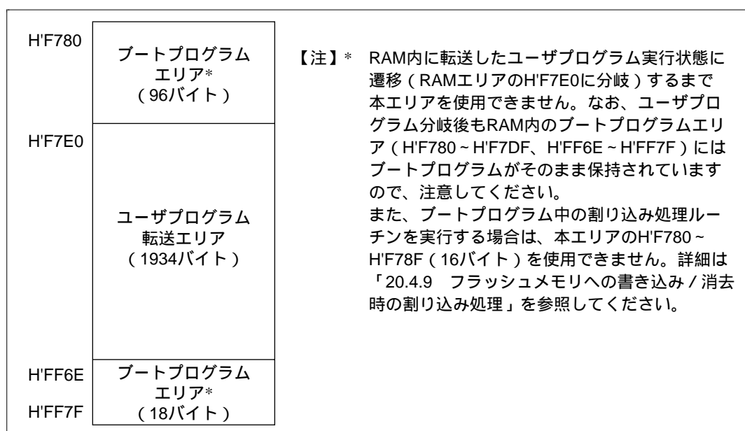
図 20.6 ブートモード時の RAM エリア
