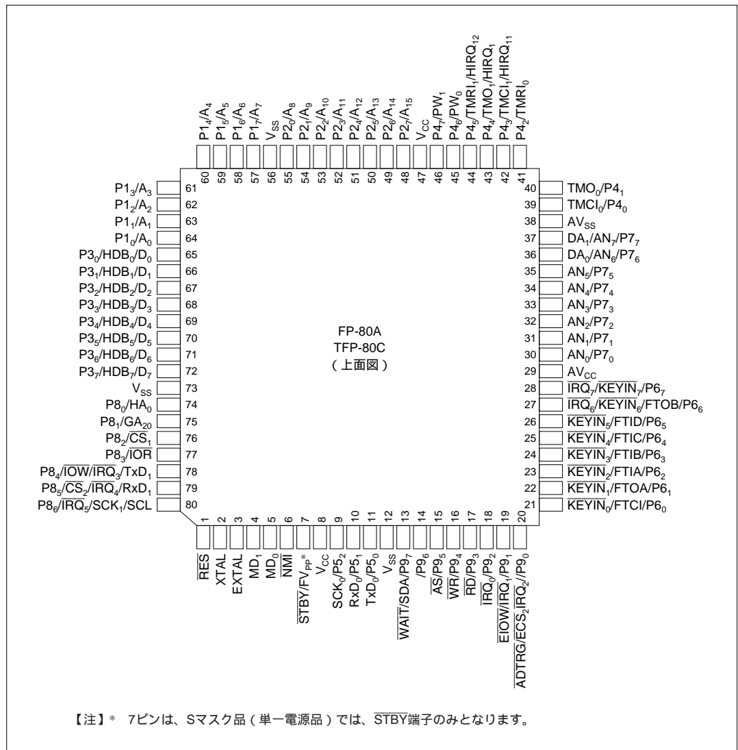
図1.2(a) H8/3337シリーズのピン配置 (FP-80A、TFP-80C : 上面図)
