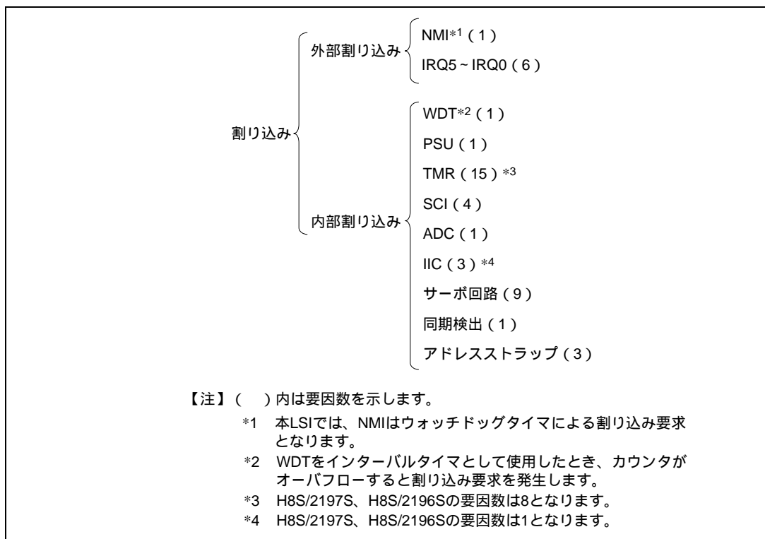
図 5.3 割り込み要因と要因数
