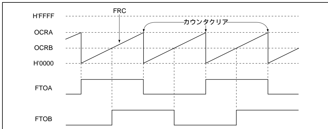
図 16.12 パルス出力例
