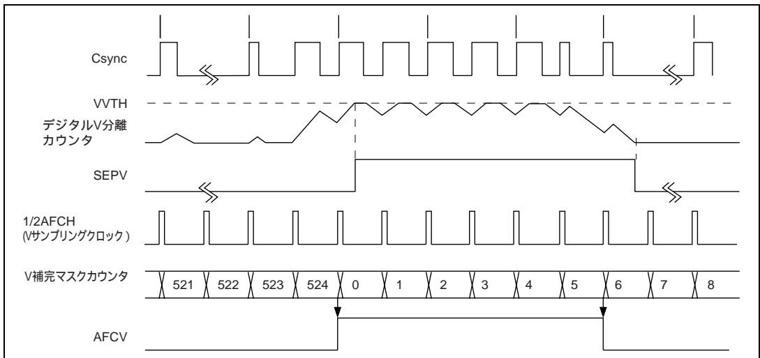
図 27.12 V 補完機能を選択した場合の AFCV 生成タイミング (NTSC の場合)
