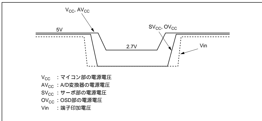
図 E.2 低消費電力モード時の電源の制御
