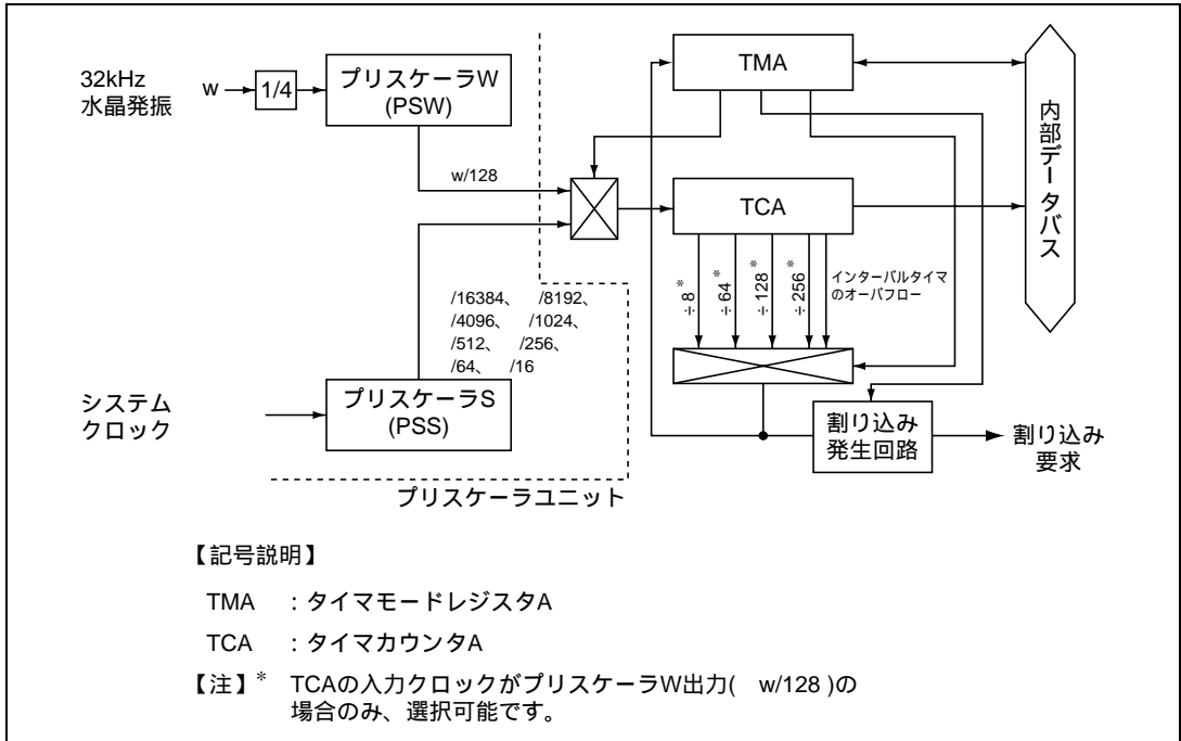
図 11.1 タイマ A ブロック図
