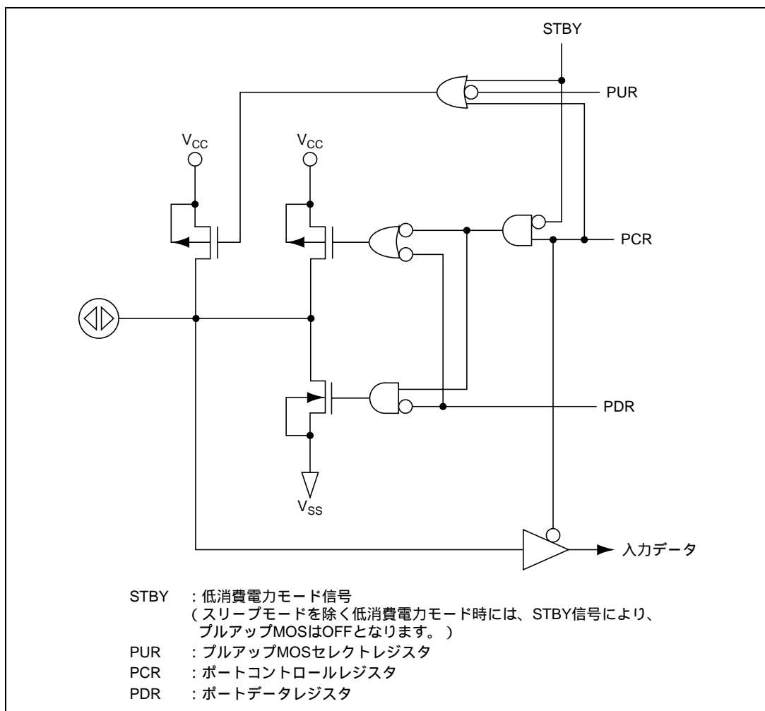
図 10.1 プルアップ MOS 付き端子の回路構成
