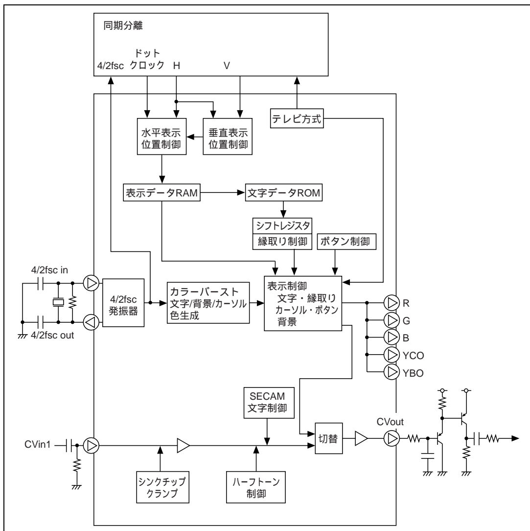
図 29.1 OSD ブロック図
