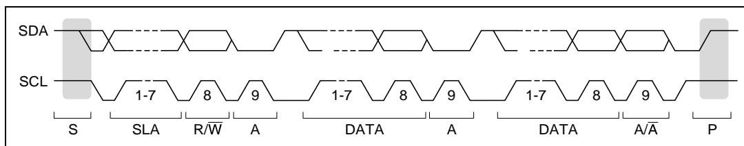
図 23.5 I 2 C バスタイミング
