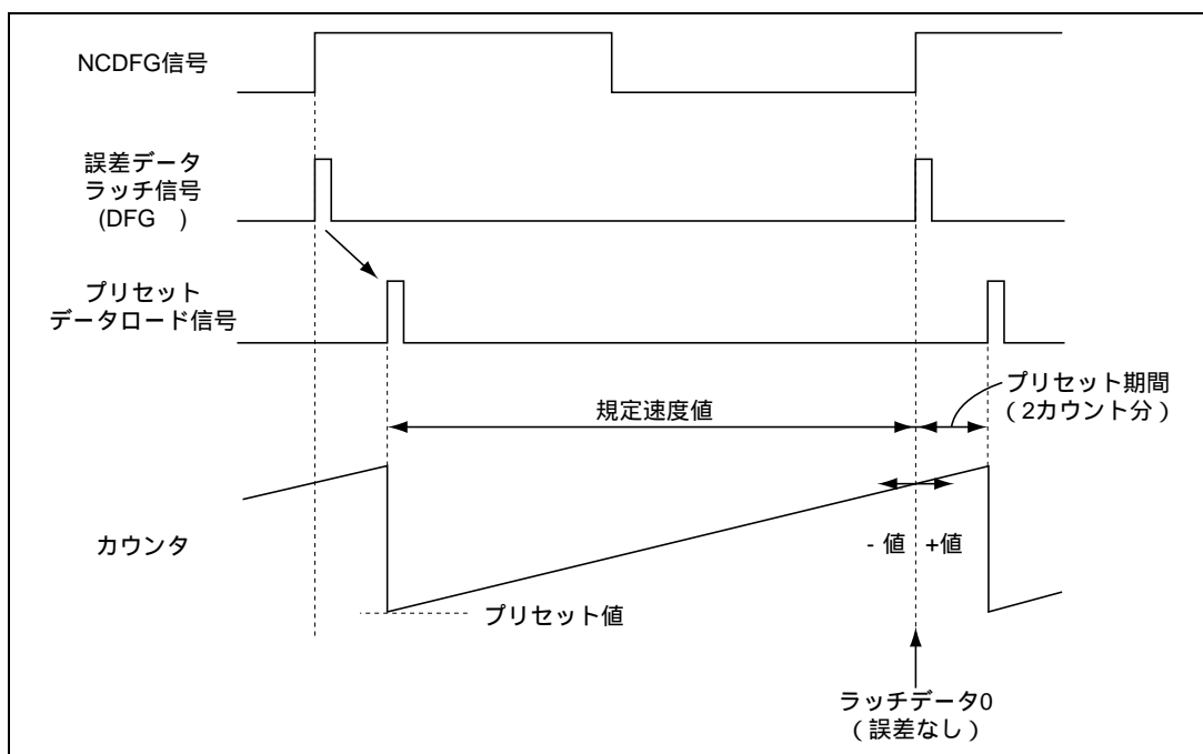
図 26.28 ドラム速度誤差検出の動作例 (DFG 立ち上がりエッジ選択)
