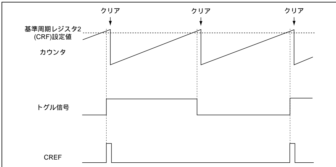
図 26.13 CREF 信号の生成
