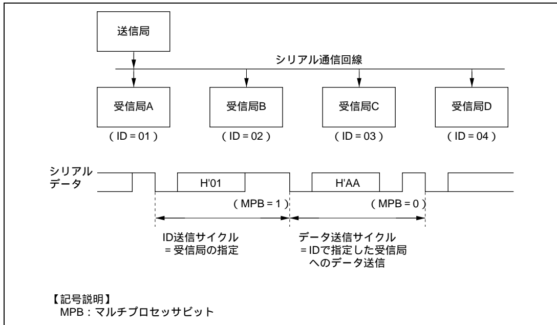
図 22.10 マルチプロセッサフォーマットを使用したプロセッサ間通信の例 (受信局 A へのデータ H'AA の送信の例)
