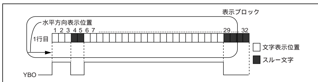
図 29.15 YBO 出力例
