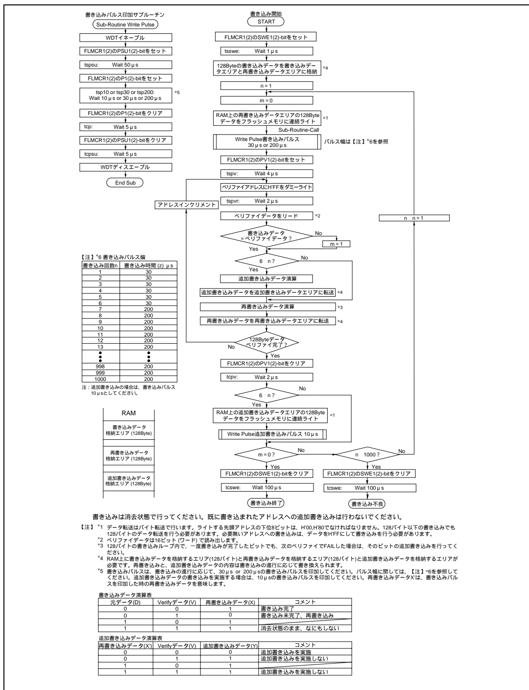
図 7.12 プログラム/プログラムペリファイフロー
