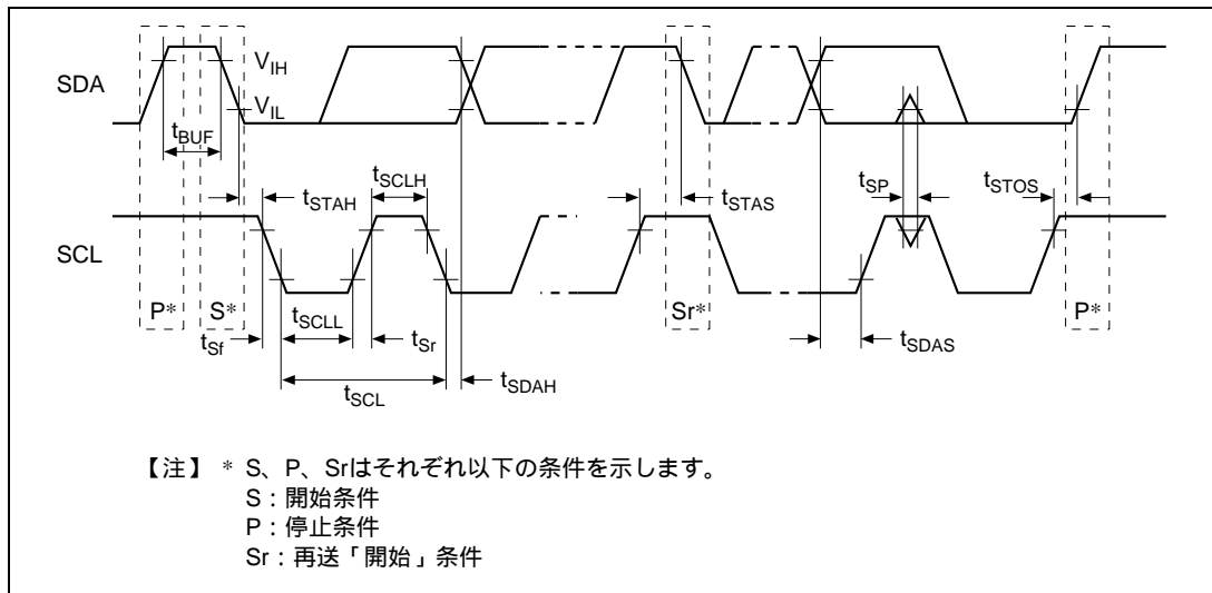
図 31.24 I 2 C バスインタフェース入出力タイミング
