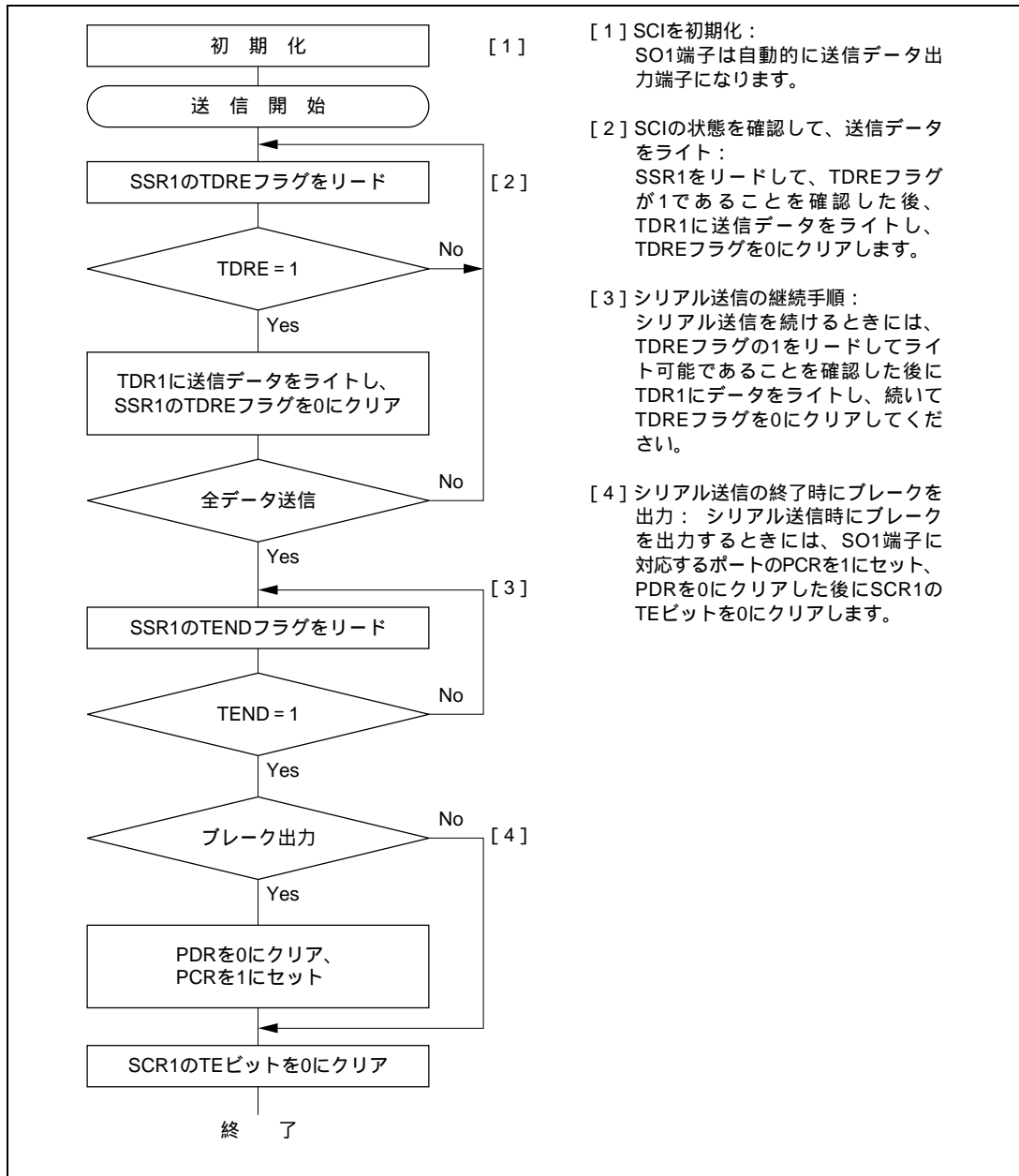
図 22.5 シリアル送信のフローチャートの例
