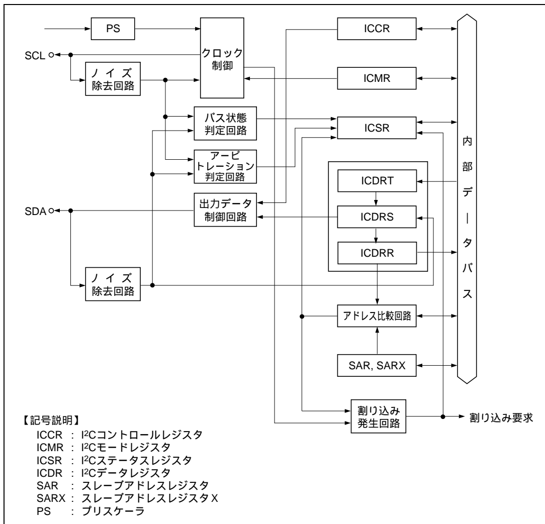
図 23.1 I 2 C バスインタフェースのブロック図
