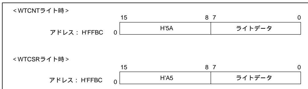
図 17.2 WTCNT、WTCSR へのライト
