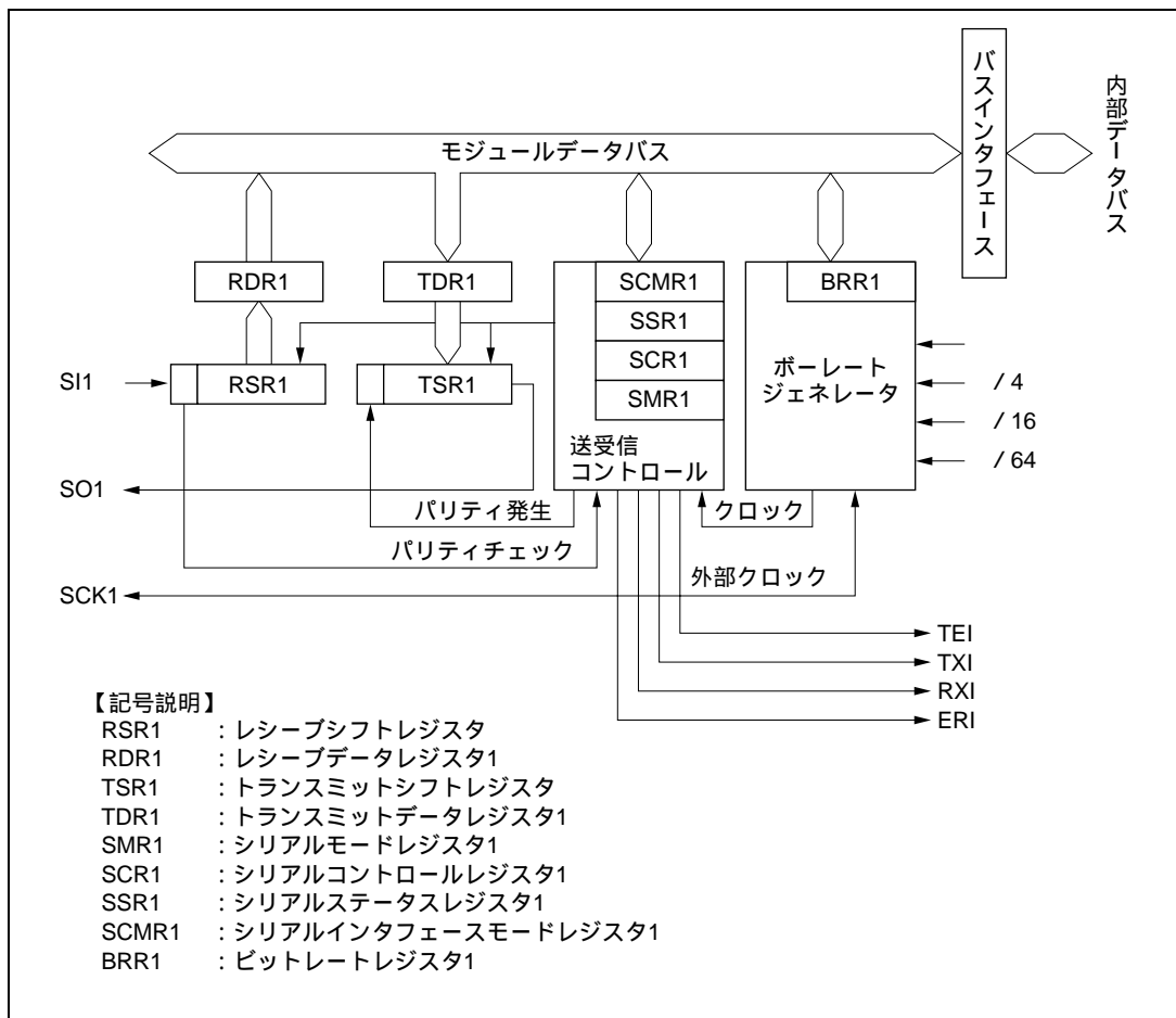
図 22.1 SCI のブロック図
