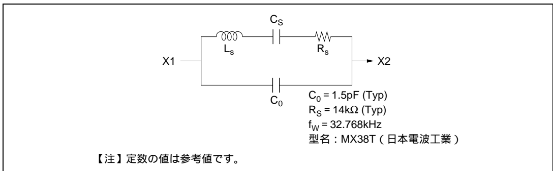
図 9.9 32.768kHz 水晶発振子の等価回路
