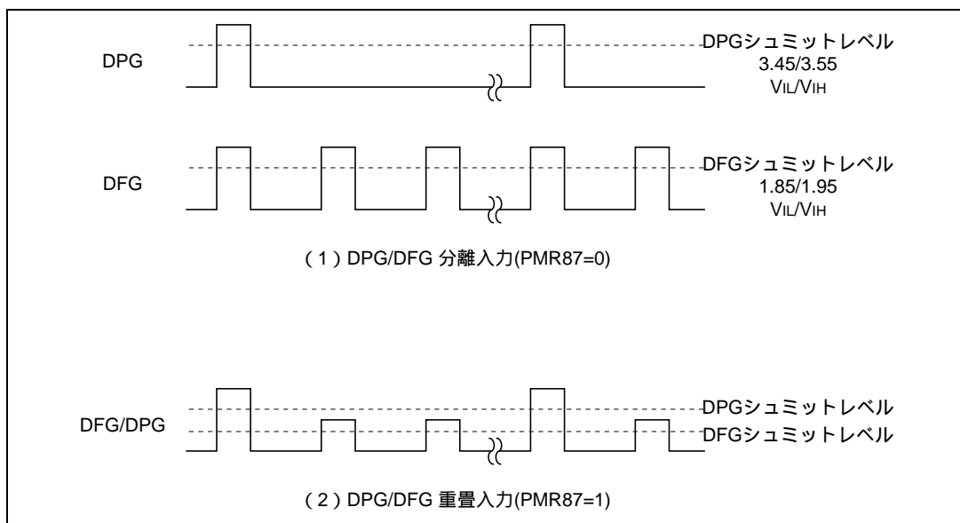
図 26.5 DFG/DPG 入力信号
