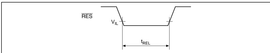
図 31.11 リセット入力タイミング
