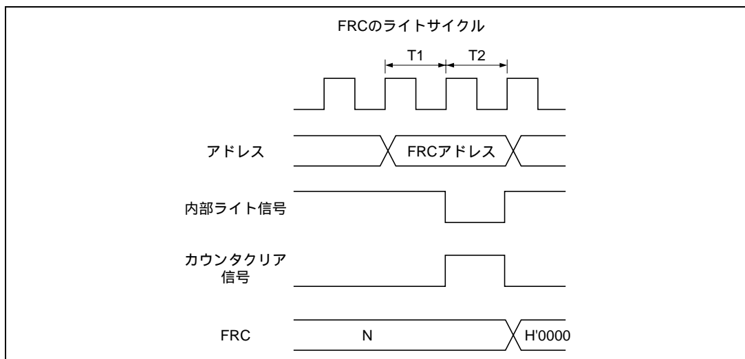
図 16.13 FRC のライトとクリアの競合
