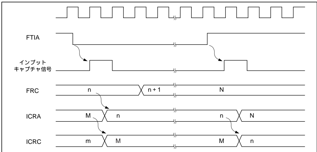
図 16.8 バッファモード時のインพุットキャプチャ信号タイミング (通常時)
