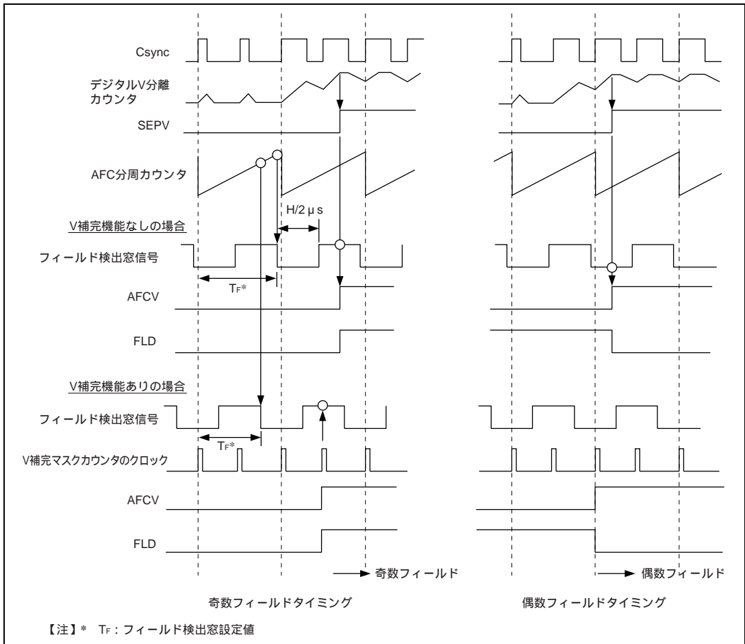
図 27.13 フィールド検出タイミング
