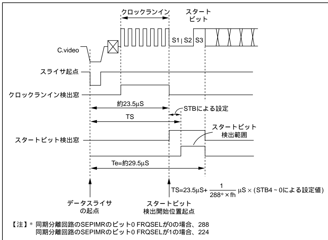
図 28.2 データスライサの起点とスタートビット検出開始位置
