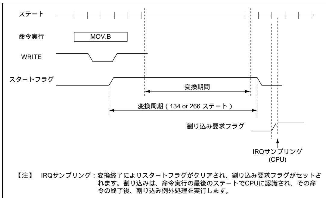
図 24.2 A/D 変換器の内部動作
