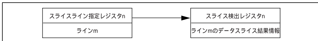
図 28.5 スライスライン指定レジスタと検出レジスタの関係
