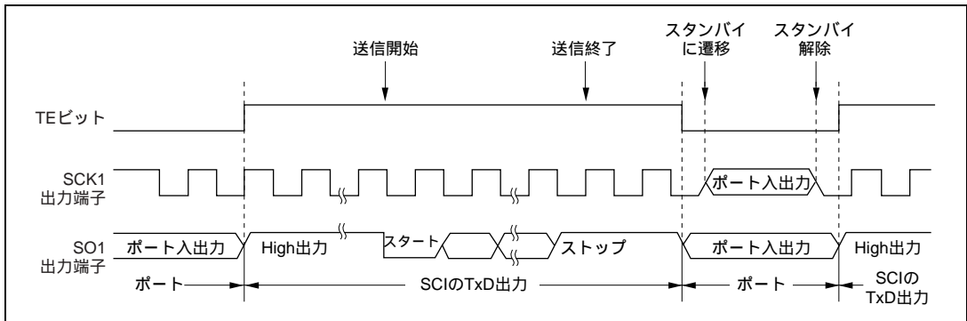
図 22.25 内部クロック、調歩同期送信の場合
