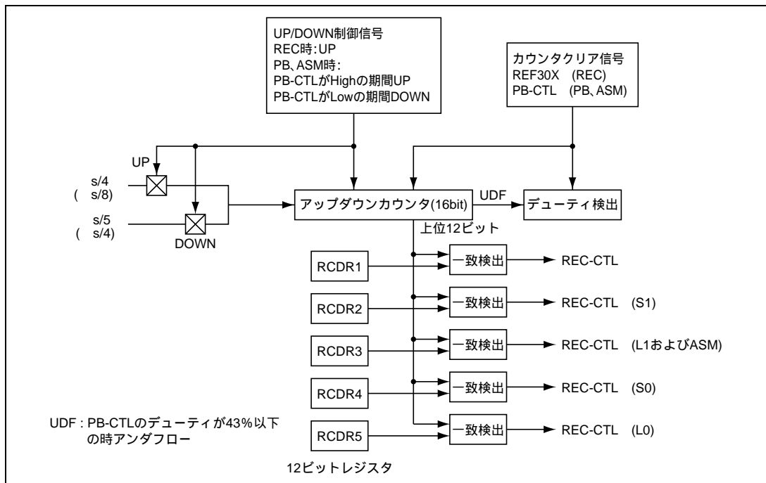
図 26.49 CTL 判別/記録回路
