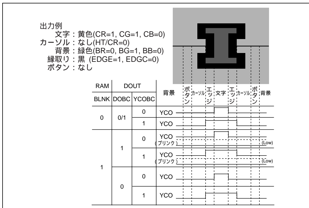
図 29.14 YCO 出力例
