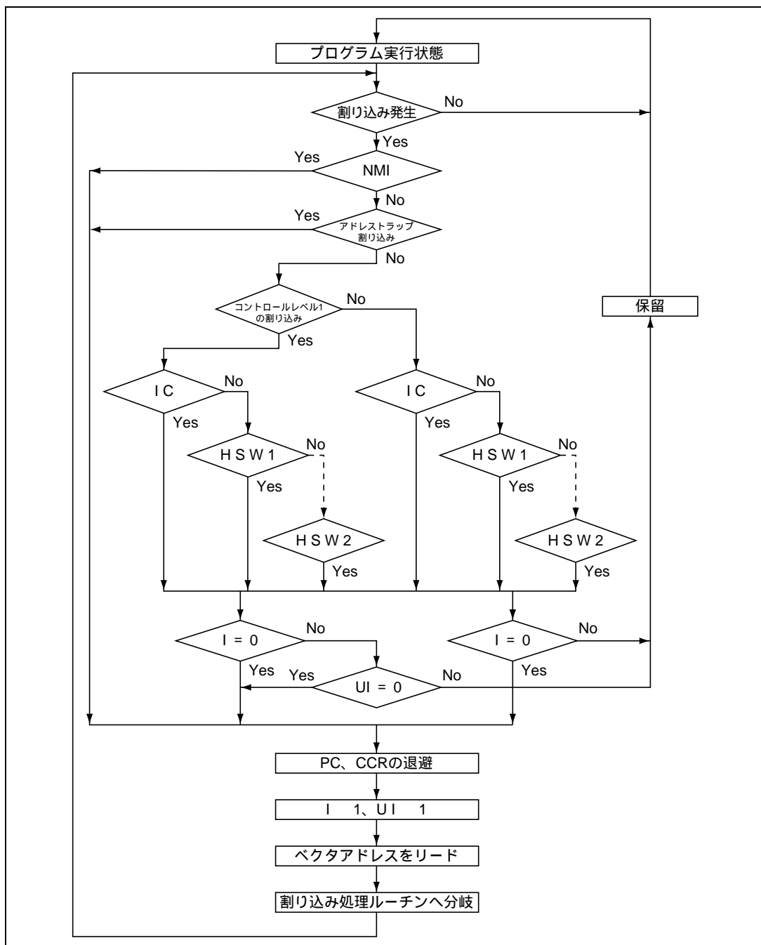
図 6.7 割り込み制御モード 1 の割り込み受けつけまでのフロー
