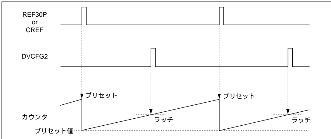
図 26.36 記録時のキャプスタン位相制御
