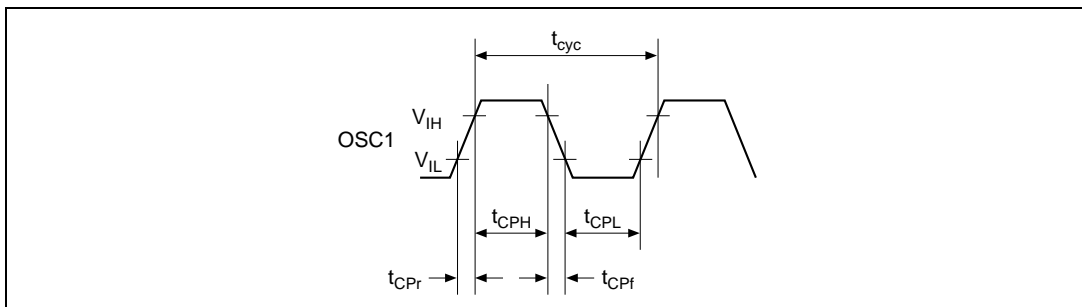
図 31.1 システムクロックタイミング
