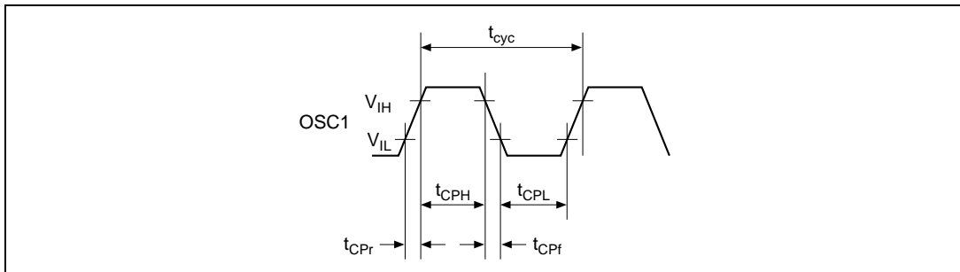
図 31.9 システムクロックタイミング
