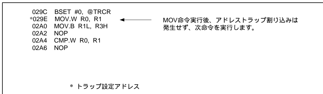
図 25.5 イネーブル
