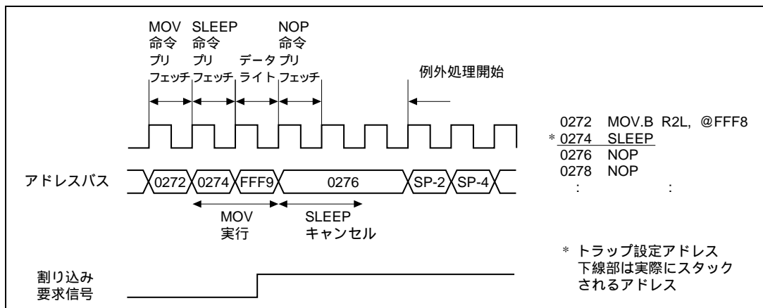
図 25.16 SLEEP 命令 (1)
