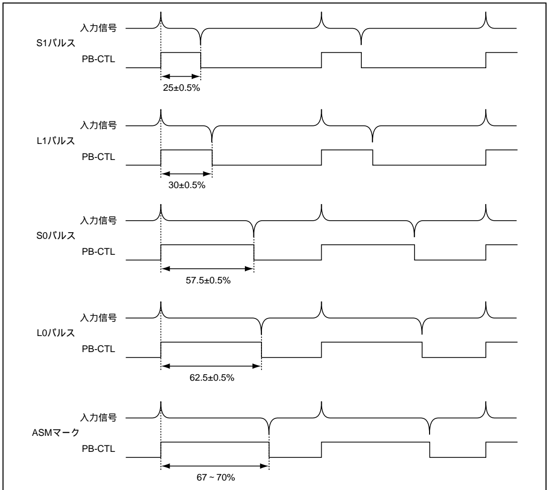
図 26.55 PB-CTL 信号のデューティ
