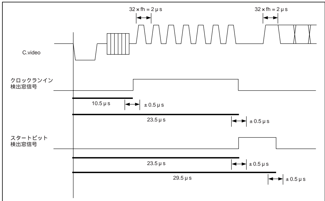
図 27.16 クロックライン検出窓信号とスタートビット検出窓信号の生成タイミング
