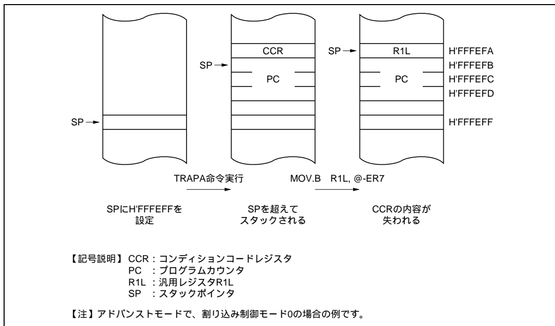
図 5.6 SP を奇数に設定したときの動作
