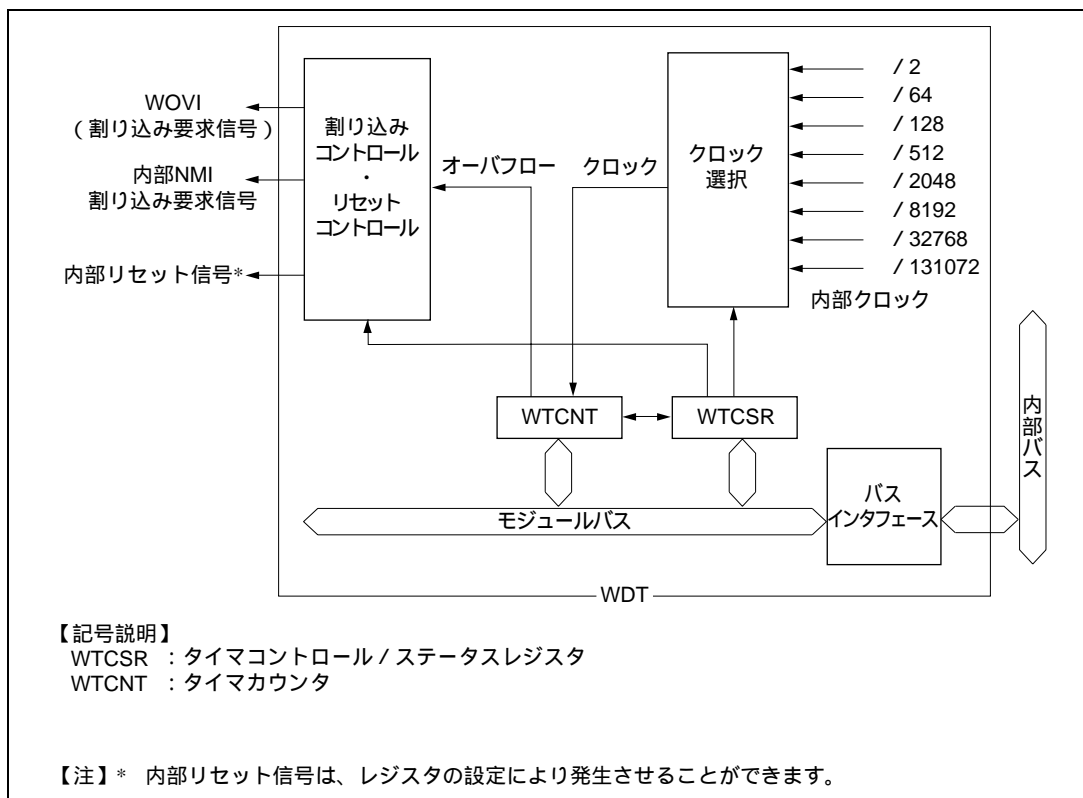
図 17.1 WDTのブロック図
