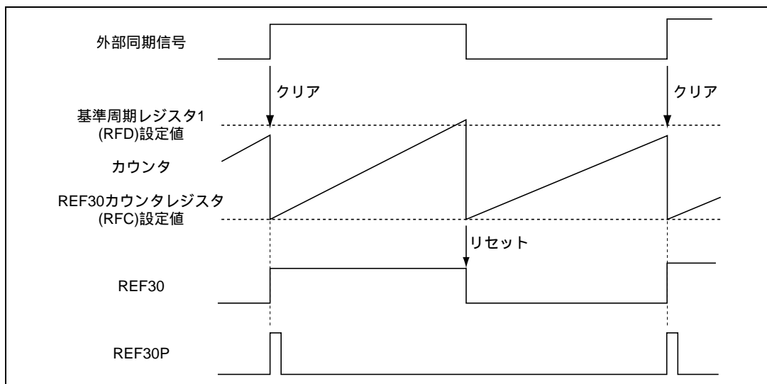
図 26.12 外部同期信号による REF30 信号
