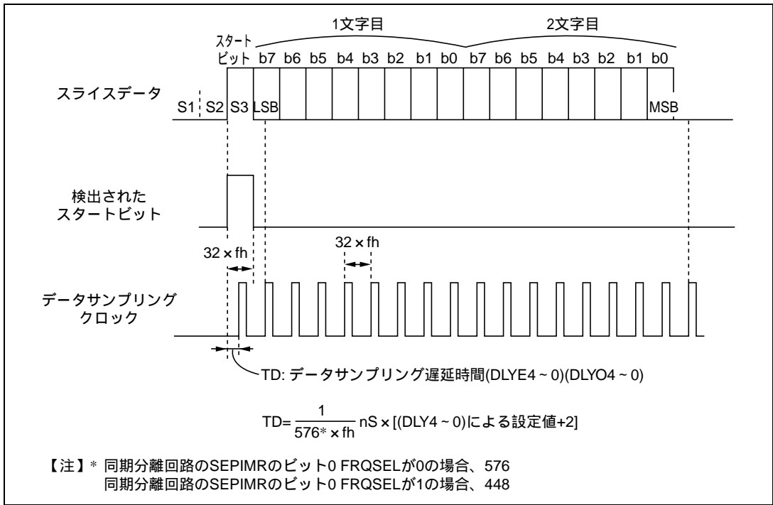
図 28.3 データサンプリングクロック説明図
