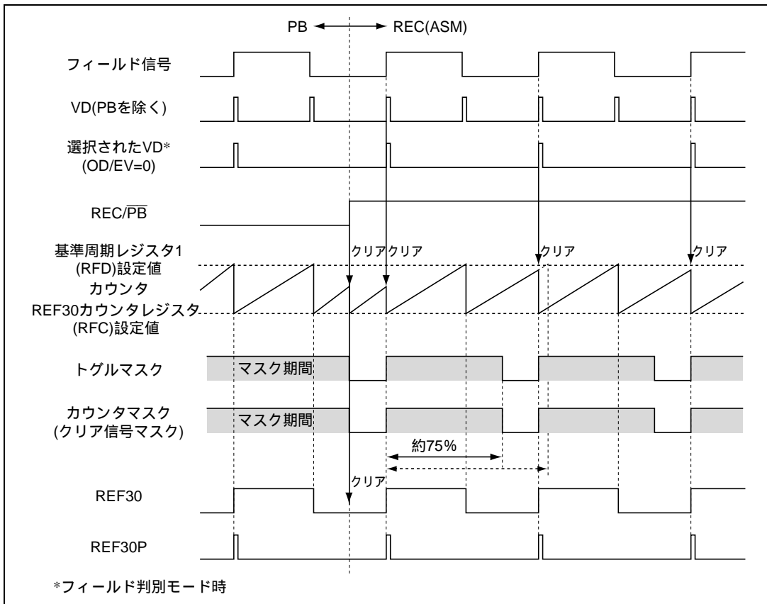
図 26.16 PB REC 切り替え時の基準信号の生成 (1)
