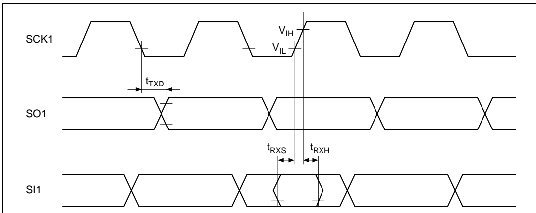
図 31.22 SCI 入出力タイミング/クロック同期式モード
