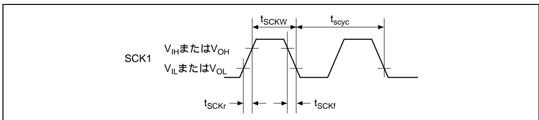
図 31.13 SCK1 クロックタイミング
