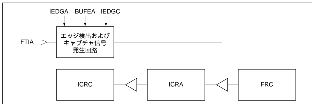
図 16.2 バッファ動作 (例)
