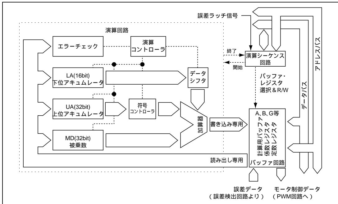
図 26.38 デジタルフィルタ演算回路ブロック図
