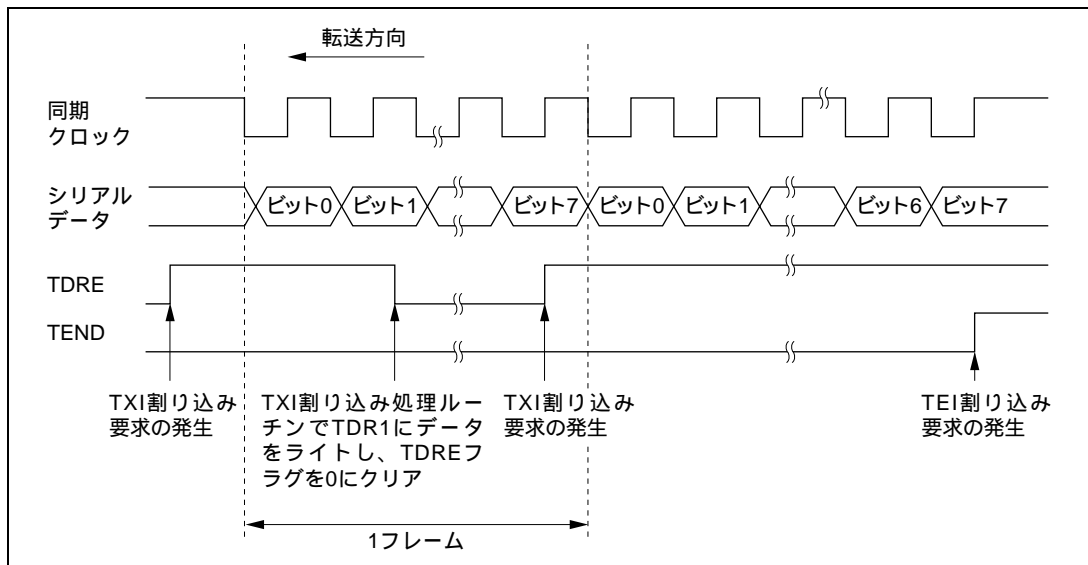
図 22.19 SCI の送信時の動作例
