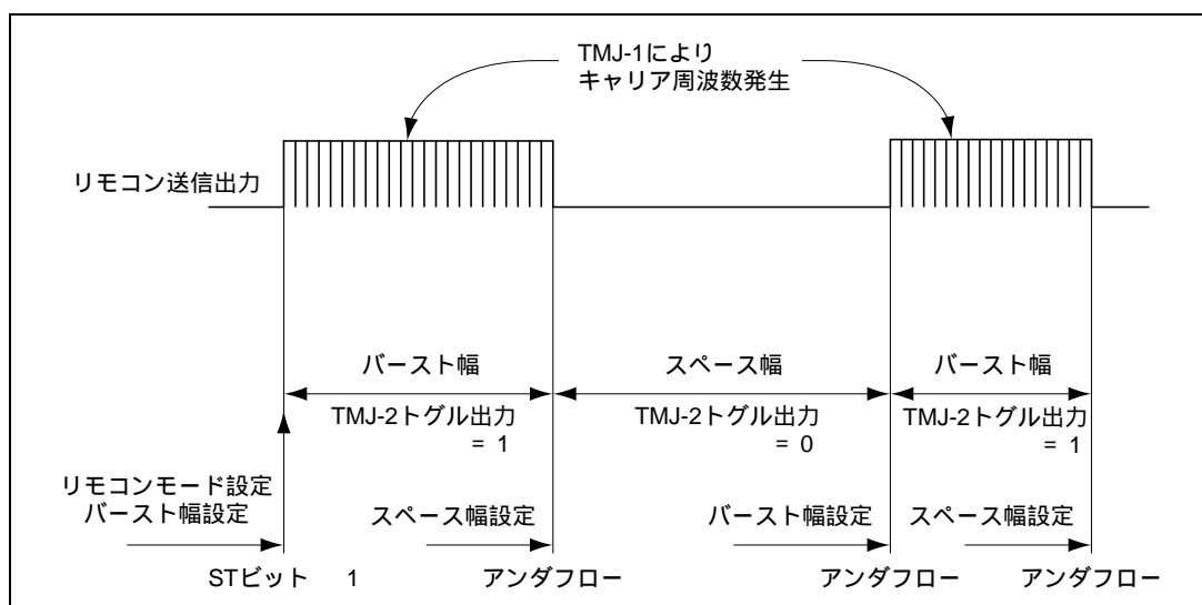
図 13.2 リモコン送信出力波形
