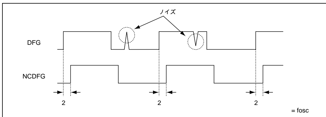
図 26.71 NCDFG 信号
