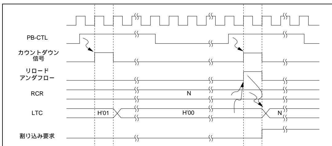
図 14.5 リロードタイミング (PB-CTL の立ち上がりエッジ選択時)
