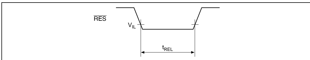
図 31.19 リセット入力タイミング
