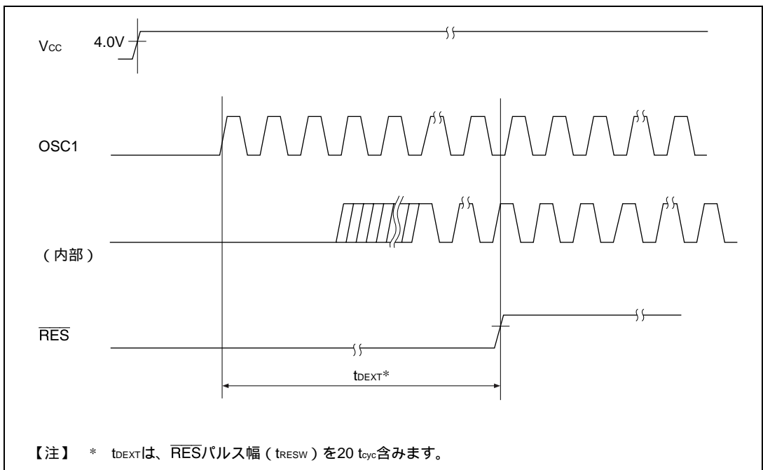
図 9.7 外部クロック安定遅延時間タイミング
