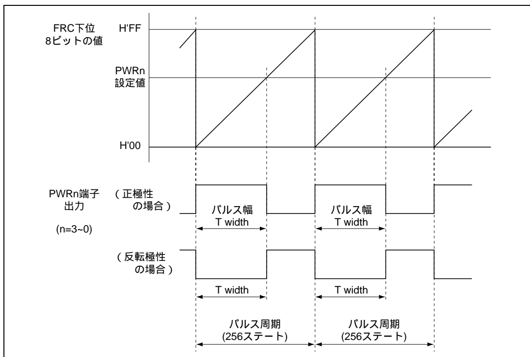
図 18.2 8ビットPWMの出力波形例
