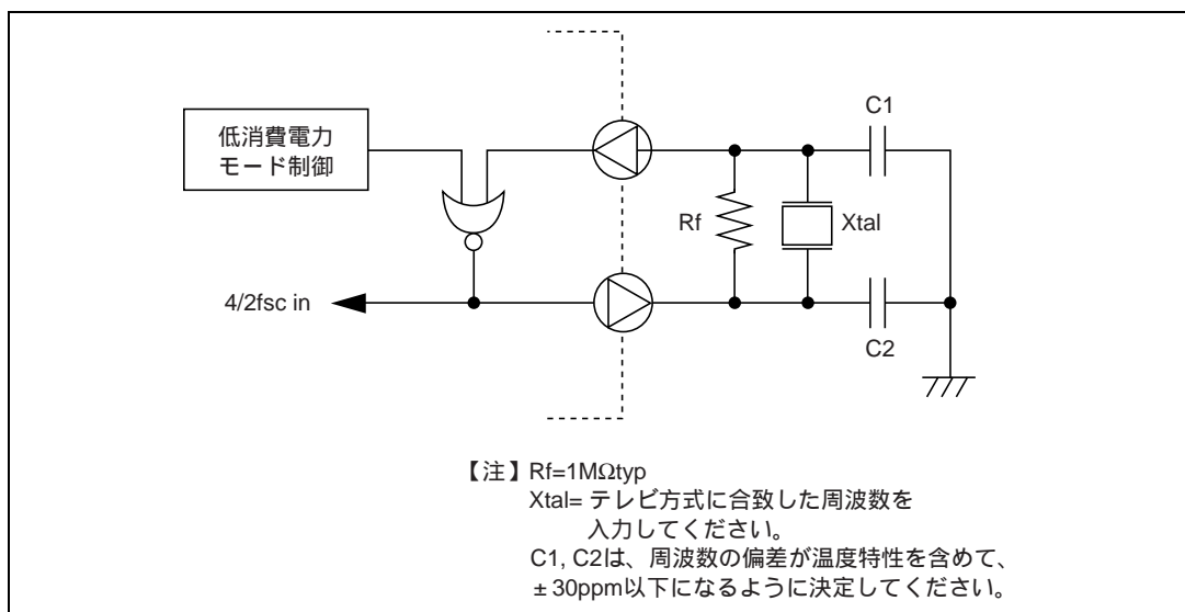
図 29.21 4/2fsc 水晶発振子の接続例
