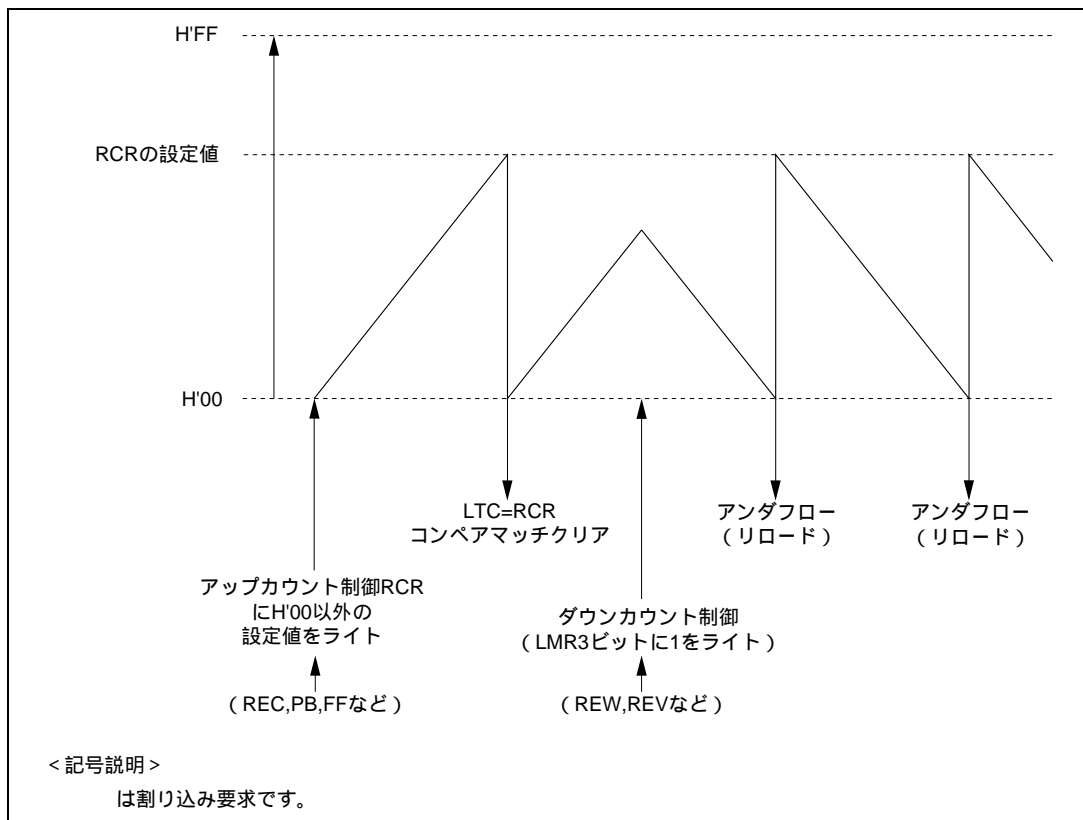
図 14.6 タイマ L の使用例
