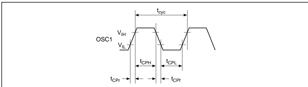
図 31.17 システムクロックタイミング
