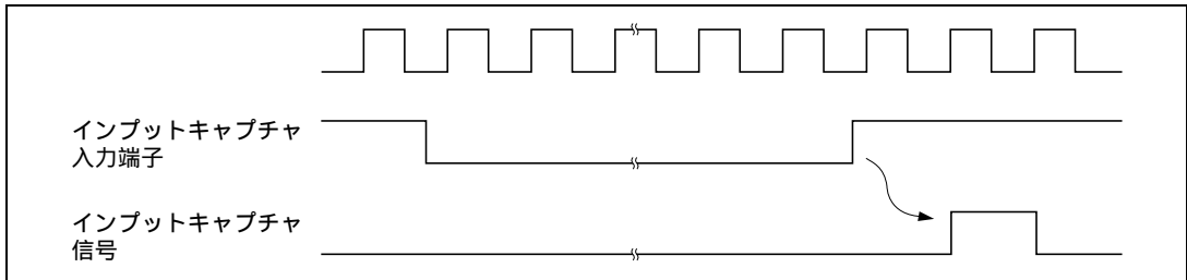
図 16.7 インพุットキャプチャ信号タイミング (通常時)
