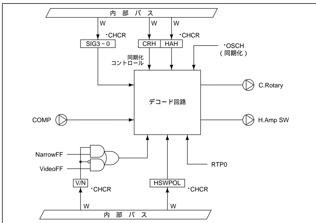
図 26.26 4ヘッド特殊再生用高速切り替え回路
