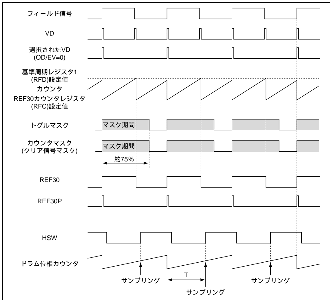
図 26.9 記録時の基準信号の生成 (正常動作)
