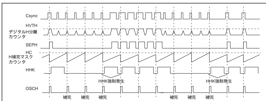
図 27.7 HHKON ビットが 1 の状態で 3 回連続補完したときの HHK 動作タイミング
