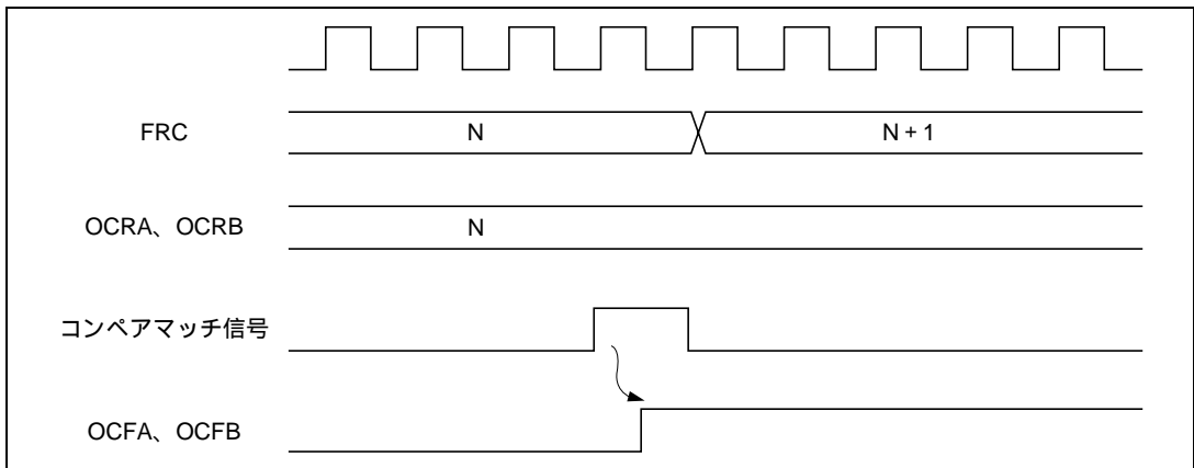
図 16.10 OCF セットタイミング
