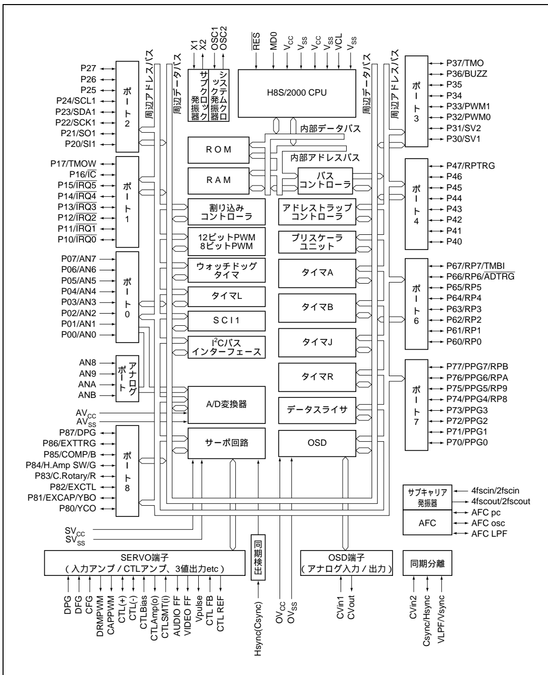
図 1.2 H8S/2197S、H8S/2196S の内部ブロック図
