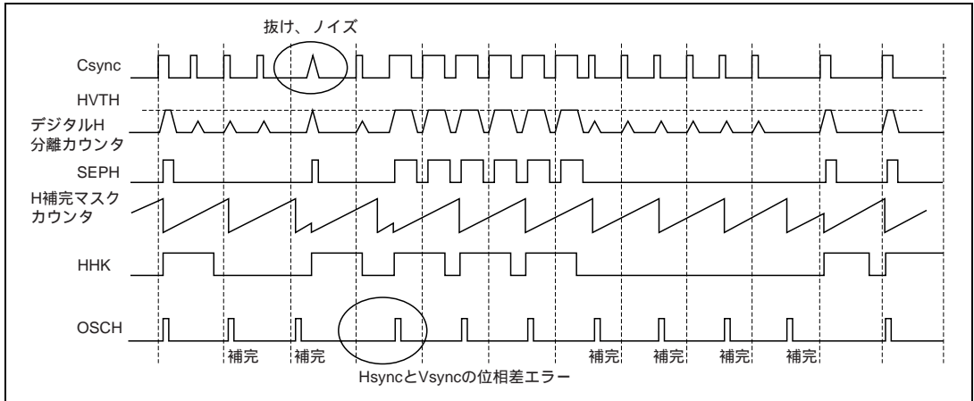
図 27.8 Hsync 位置にある等価パルス無入力後のノイズ発生による Hsync と Vsync の位相差エラー発生タイミング
