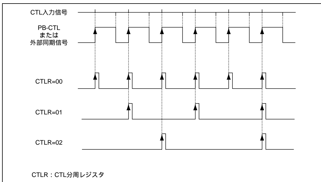
図 26.64 CTL 分周波形
