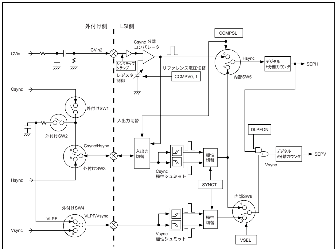
図 27.2 同期分離入力の選択回路図
