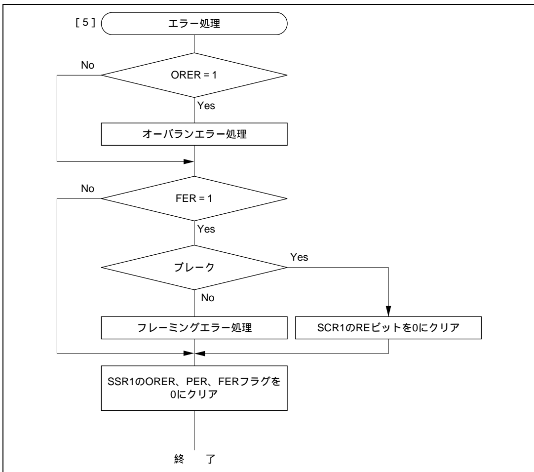
図 22.14 マルチプロセッサシリアル受信のフローチャートの例 (2)
