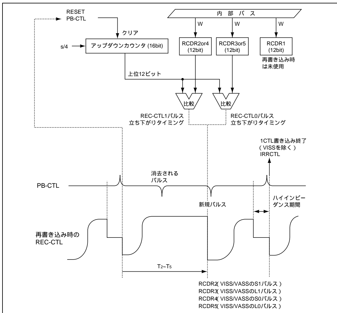
図 26.62 再書き込み時の REC-CTL と RCDR2 ~ 5 の関係
