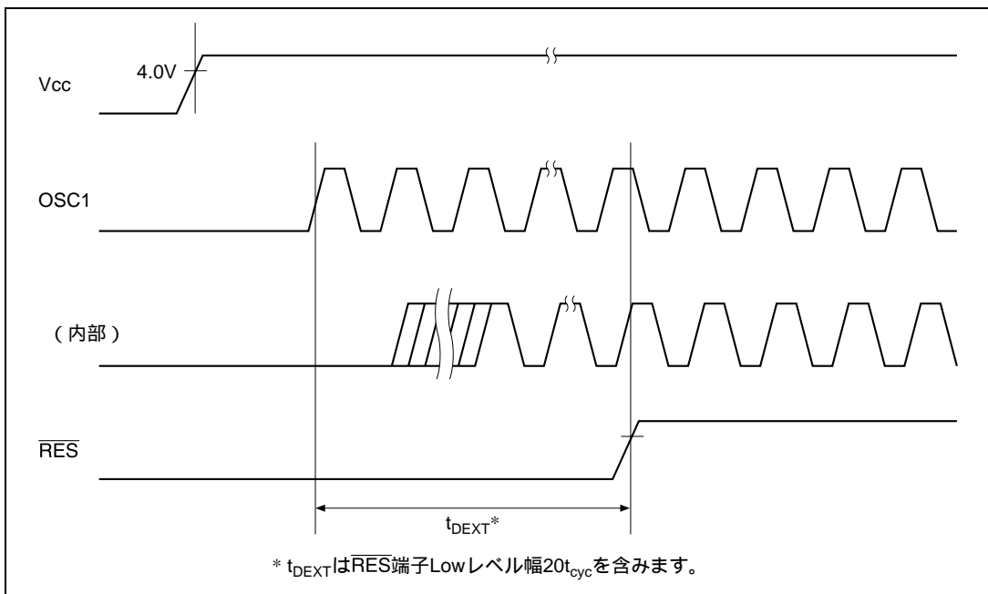
図 31.10 外部クロック安定遅延時間タイミング
