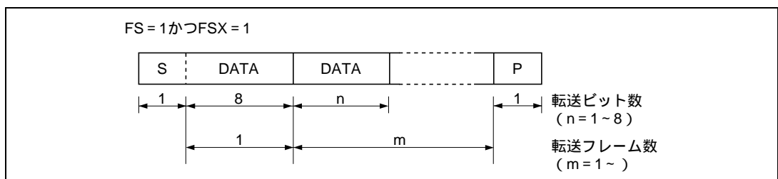
図 23.4 I 2 C バスデータフォーマット (シリアルフォーマット)
