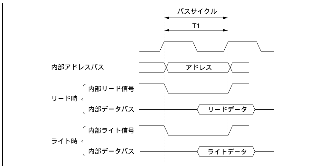
図 2.18 内蔵メモリアクセスサイクル
