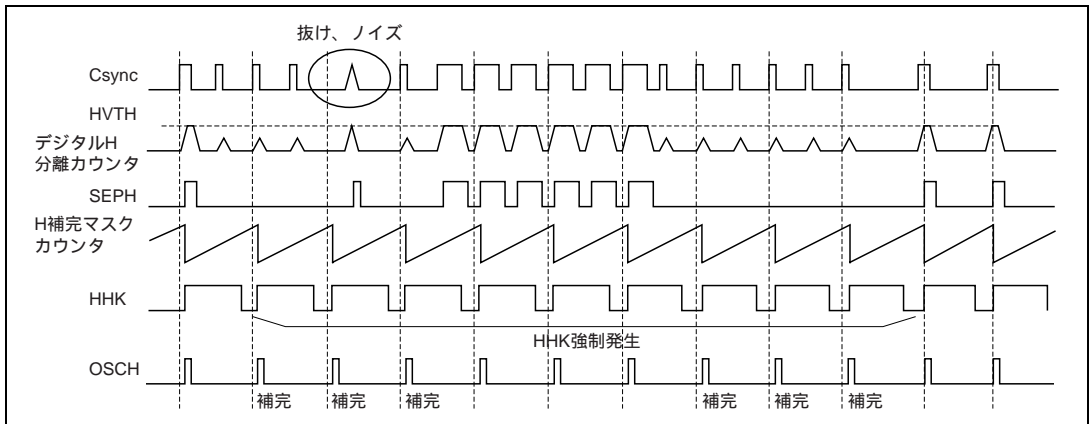
図 27.9 等化パルス未検出時の V ブランキング期間の HHK 強制動作タイミング
