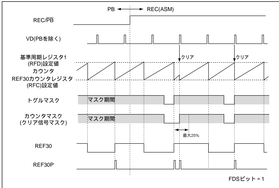
図 26.21 RFD ビット = 1 の時、PB REC 切り替え時の基準信号の生成 (4)
