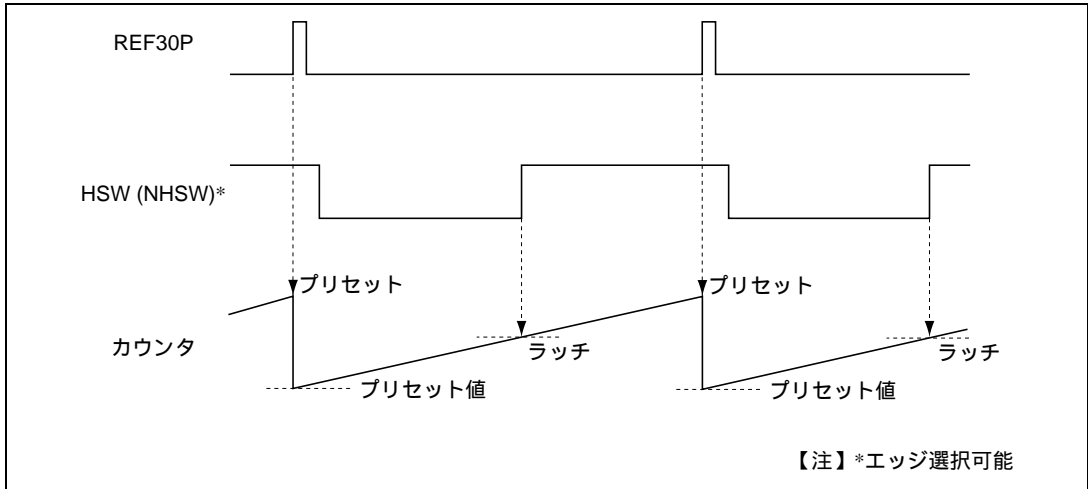
図 26.30 再生時のドラム位相制御 (HSW 立ち上がりエッジを選択)
