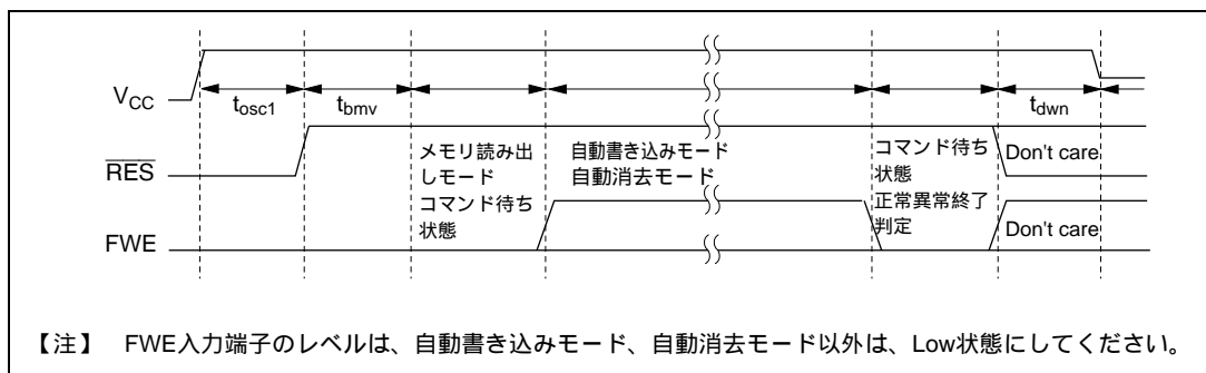
図 7.23 発振安定時間とブートプログラム転送時間、電源立ち下げシーケンス
