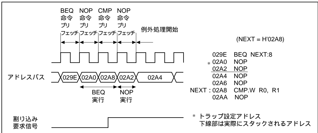
図 25.7 Bcc 命令で条件不成立時 (8 ビットディスプレイースメント)
