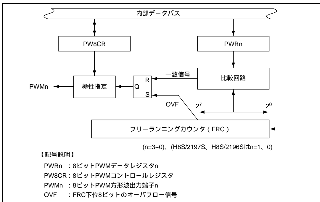
図 18.1 8ビットPWMのブロック図(1チャンネル分)
