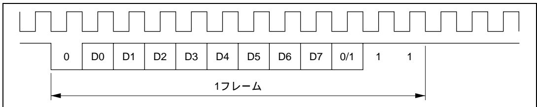
図 22.3 出力クロックと通信データの位相関係 (調歩同期式モード)
