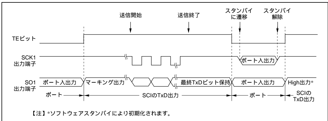
図 22.26 内部クロック、クロック同期送信の場合
