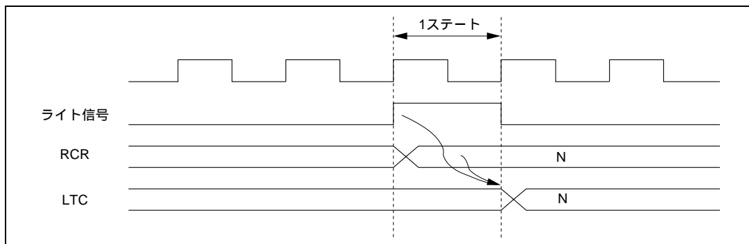
図 14.4 RCR ライト、リロードタイミング
