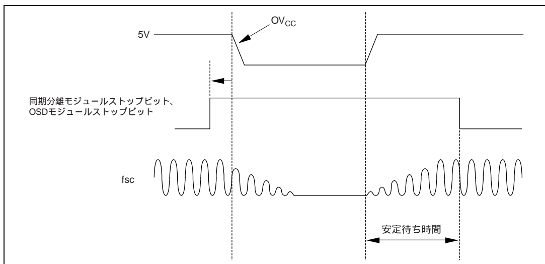
図 E.3 OV_{CC} の立ち上げ・立ち下げ時のモジュールストップビットの設定順序
