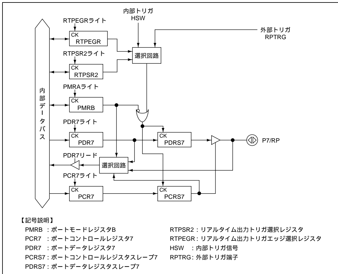
図 10.3 ポート7の機能ブロック図
