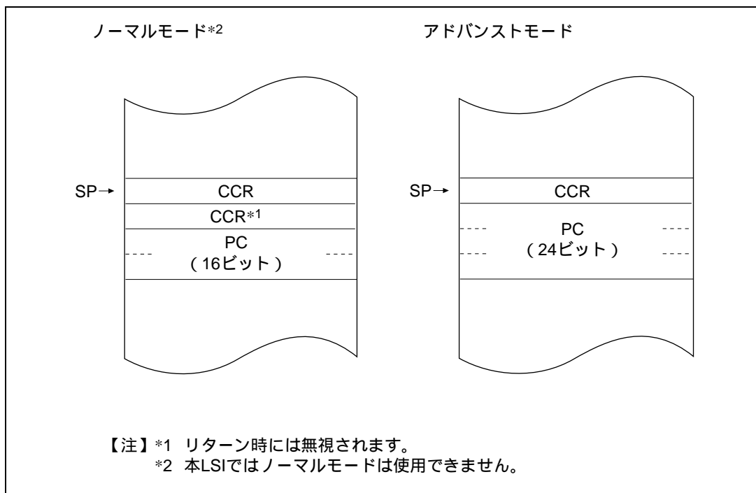
図 2.17 例外処理終了後のスタックの状態 (例)
