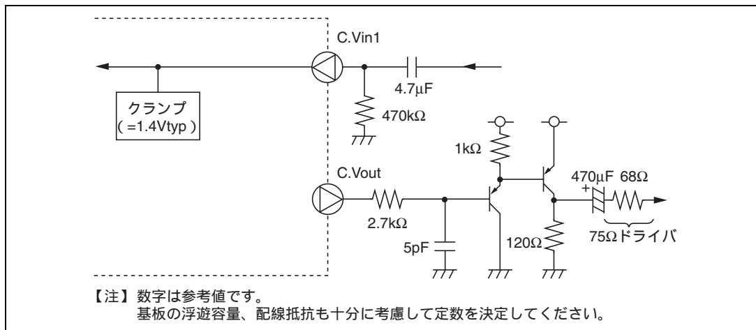
図 E.7 OSD 部 外部回路例
