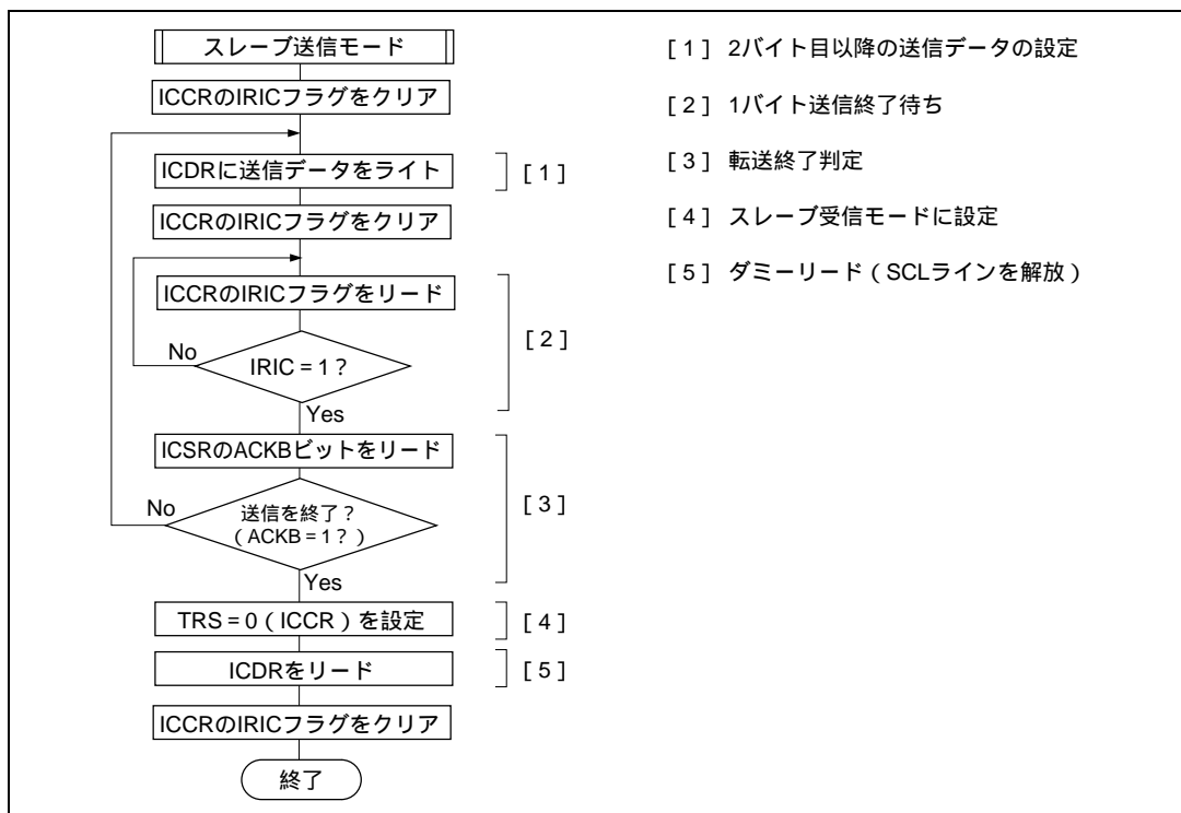
図 23.17 スレーブ送信モードフローチャート例
