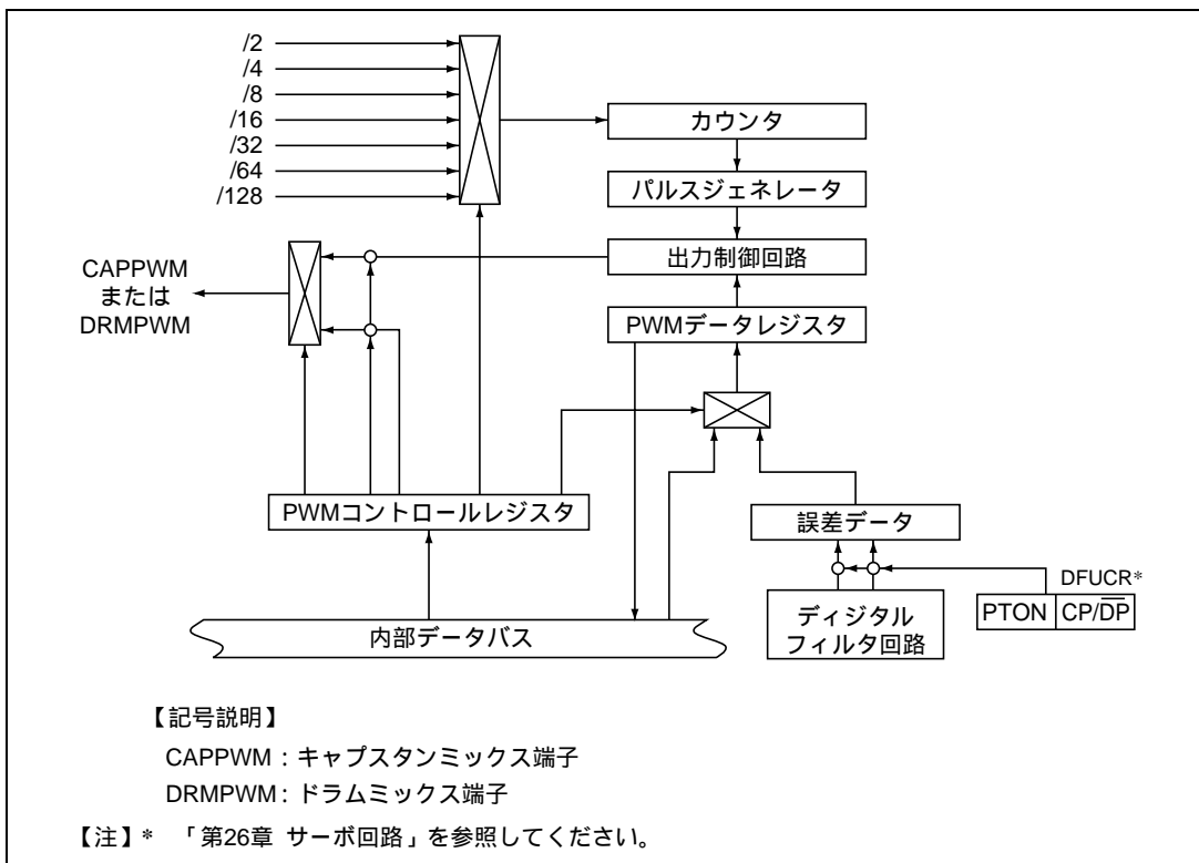
図 19.1 12ビット PWM のブロック図 (1チャンネル分)
