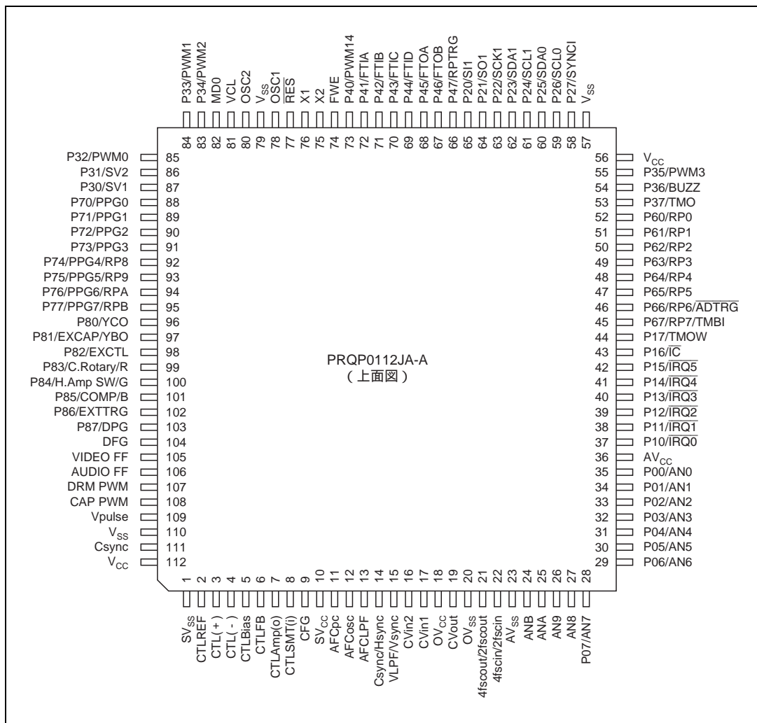
図 1.3 ピン配置図 (H8S/2197S、H8S/2196S を除く)
