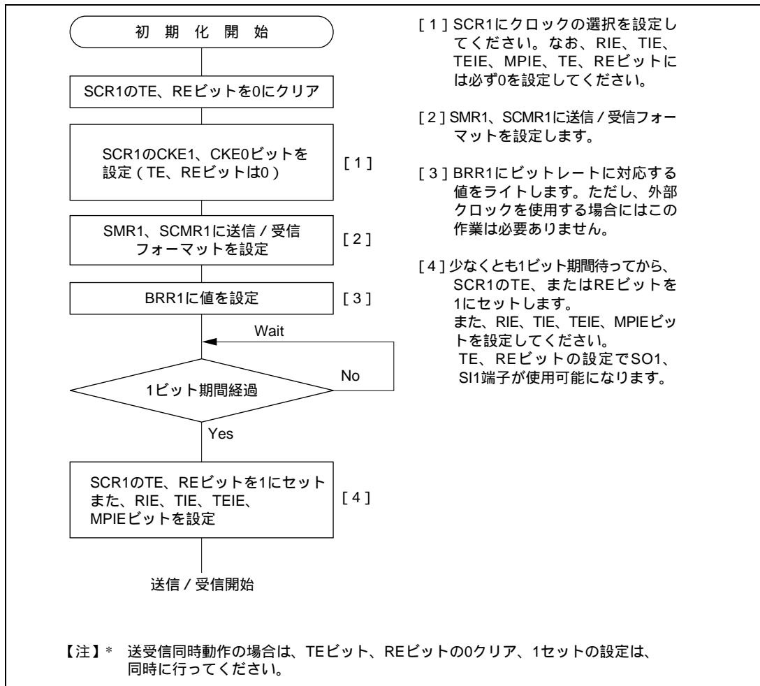
図 22.17 SCI の初期化フローチャートの例
