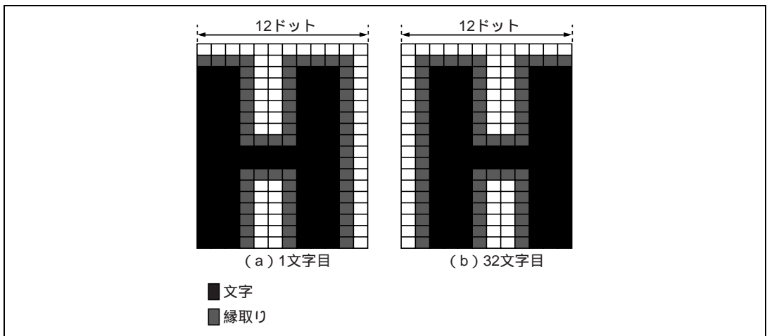
図 29.18 行の表示開始および最終番地の文字例
