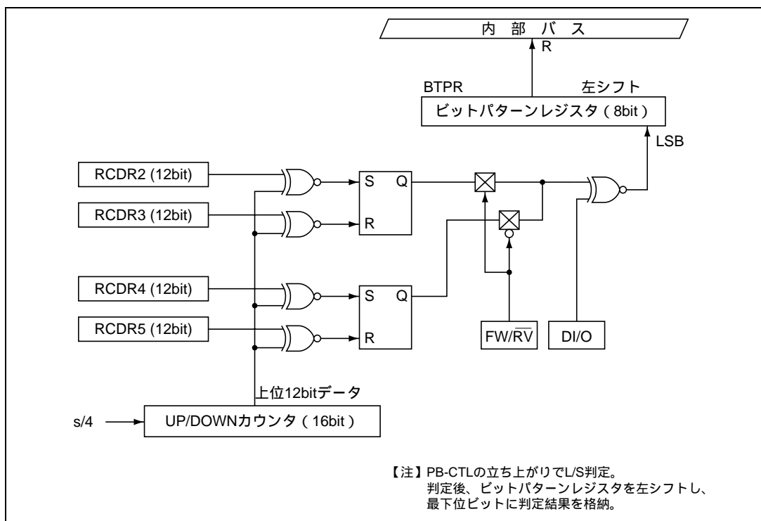
図 26.59 Long/Short パルス検出
