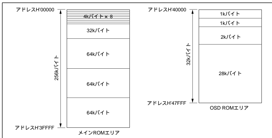
図 7.6 フラッシュメモリのブロック分割
