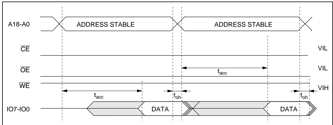
図 7.18 \overline{CE} 、 \overline{OE} イネーブル状態リード時のタイミング波形
