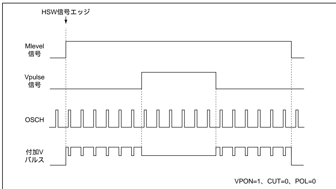
図 26.46 負極を指定したときの付加Vパルス
