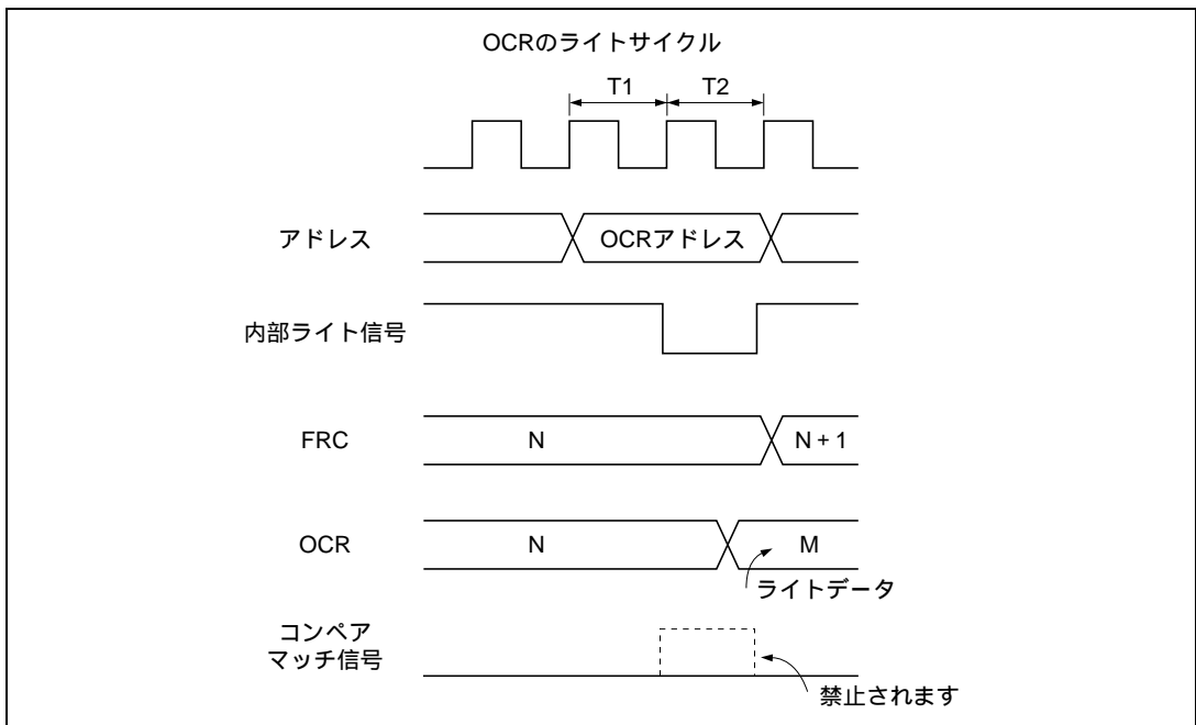
図 16.15 OCR とコンペアマッチの競合
