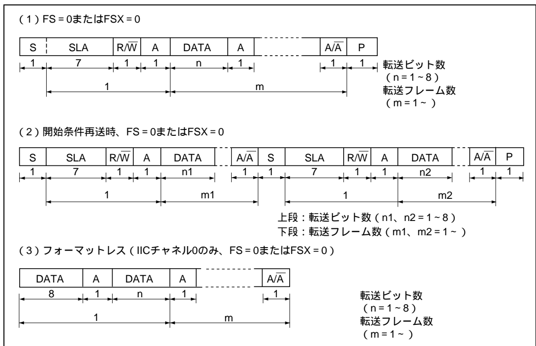
図 23.3 I 2 C バスデータフォーマット (I 2 C バスフォーマット)
