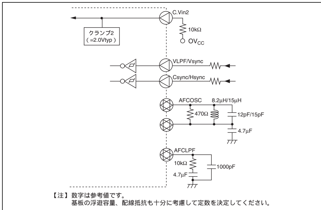
図 E.10 同期分離・データスライサ部の外部回路例 ( (3)Hsync、Vsync 分離入力 )
