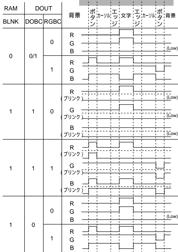
図 29.12 RGB 出力例 ( 1 )
