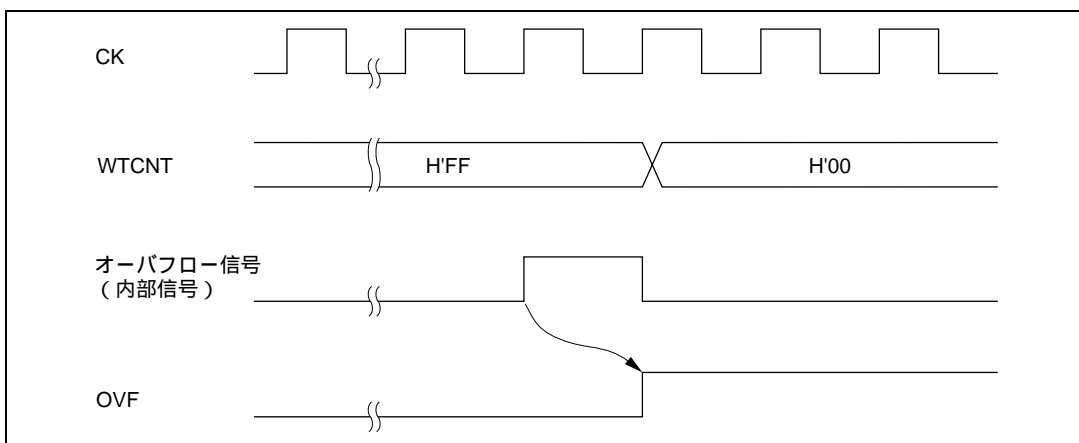
図 17.5 OVF のセットタイミング
