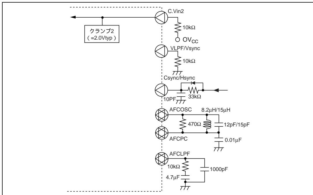
図 E.9 同期分離・データスライサ部の外部回路例 (2)Csync からの同期分離)
