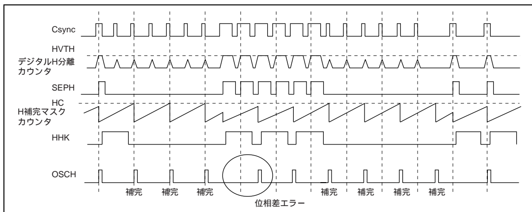
図 27.6 等価パルス未検出時の Hsync と Vsync の位相差エラー発生タイミング
