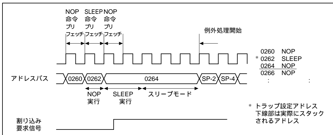
図 25.17 SLEEP 命令 (2)
