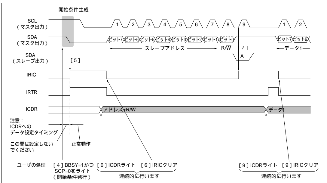
図 23.6 マスタ送信モード動作タイミング例 (MLS = WAIT = 0 のとき)
