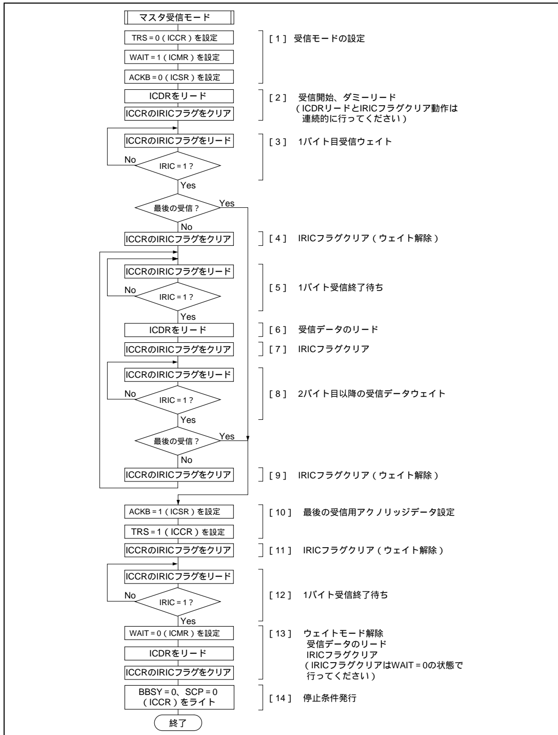
図 23.15 マスタ受信モードのフローチャート例
