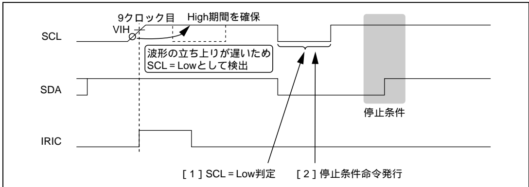
図 23.20 停止条件発行タイミング
