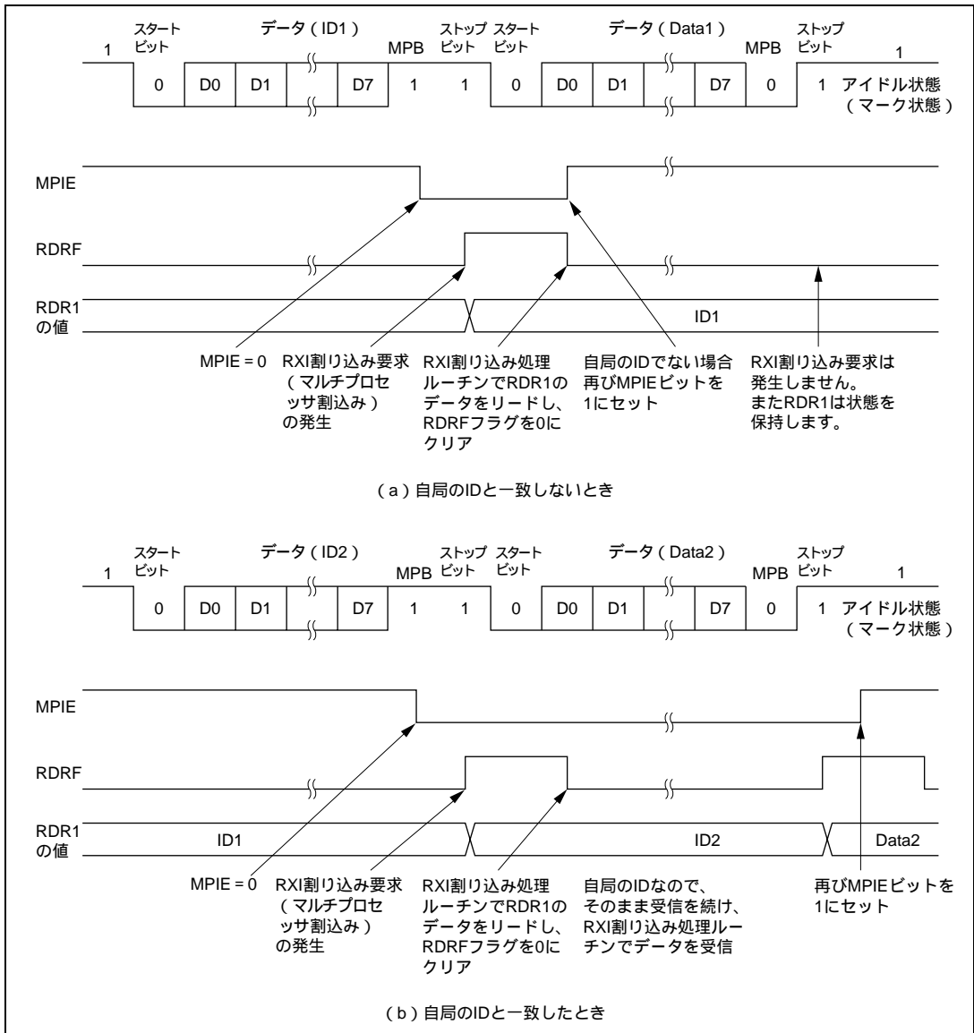
図 22.15 SCI の受信時の動作例 (8ビットデータ/マルチプロセッサビットあり/1ストップビットの例)
