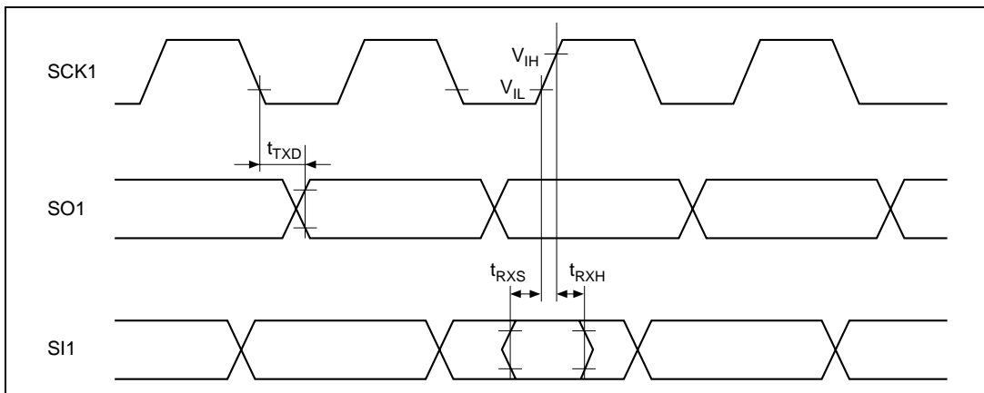
図 31.6 SCI 入出力タイミング/クロック同期式モード
