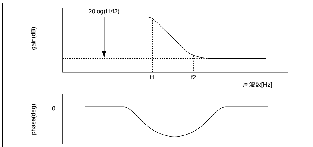
図 26.41 ラグリードフィルタの周波数特性
