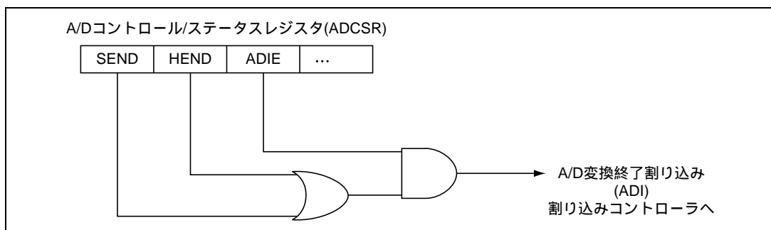
図 24.4 A/D 変換終了割り込みブロック図
