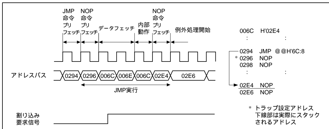
図 25.14 JMP 命令 (メモリ間接)
