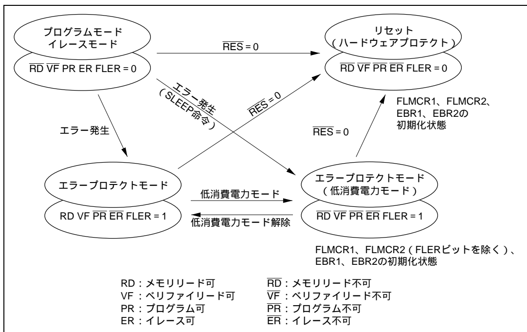
図 7.14 フラッシュメモリの状態遷移図
