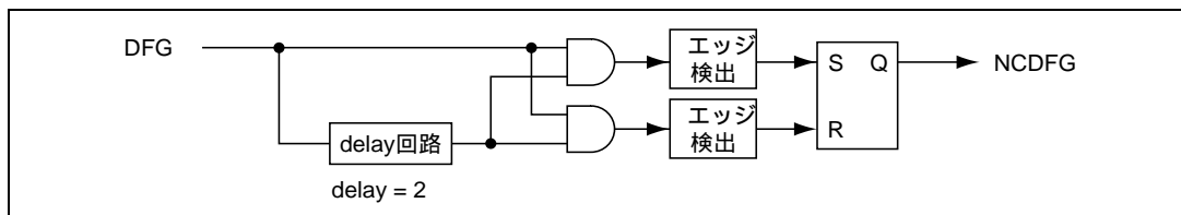
図 26.70 DFG ノイズ除去回路
