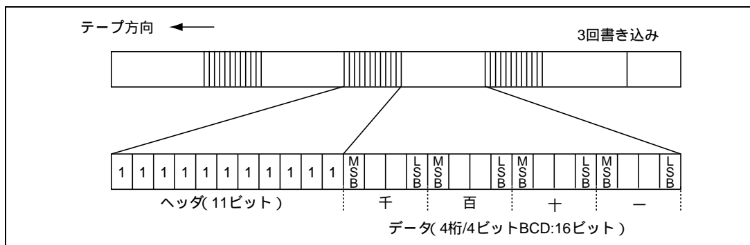
図 26.58 VASS (INDEX) のフォーマット
