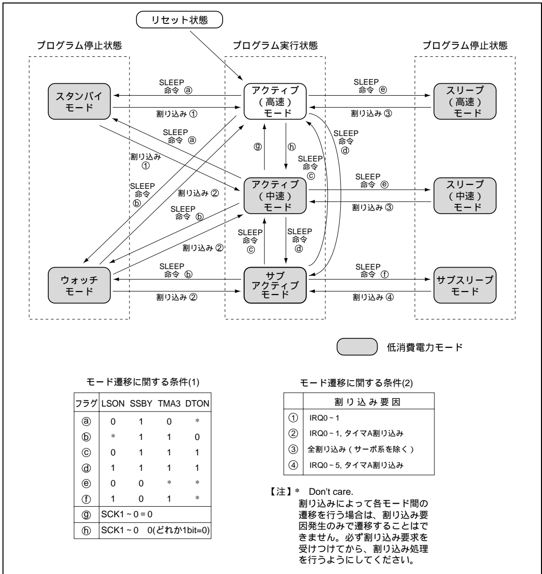
図 4.1 モード遷移
