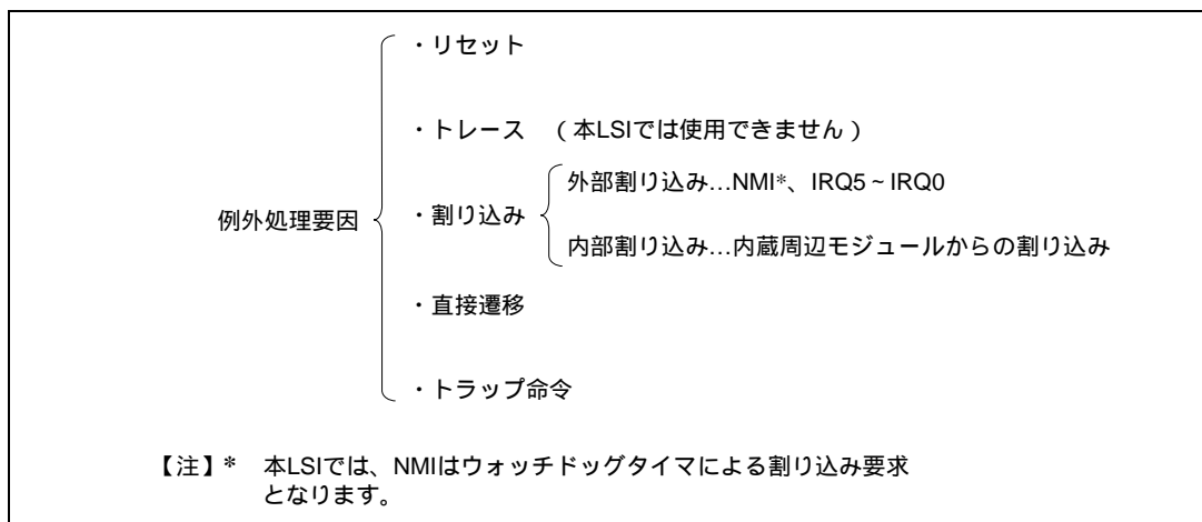
図 5.1 例外処理要因
