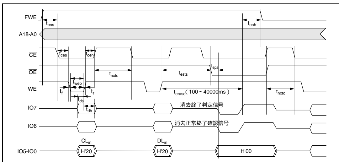
図 7.21 自動消去モードのタイミング波形
