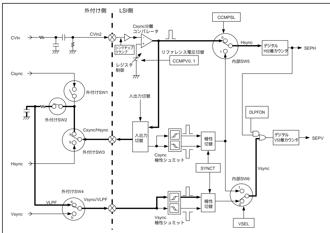
図 27.17 Cvin2 入力 で Vsync シュミット を使用 した 場合 の 分離 入力
