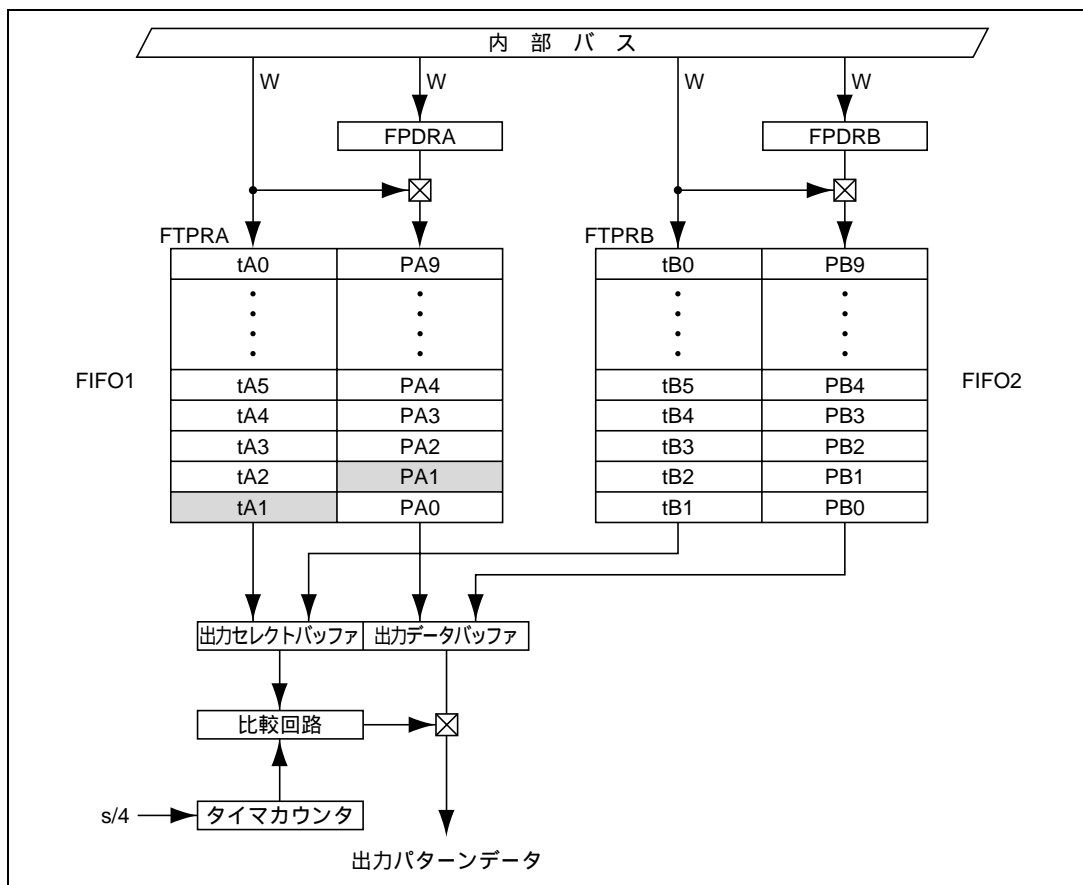
図 26.24 HSW タイミング生成回路動作例
