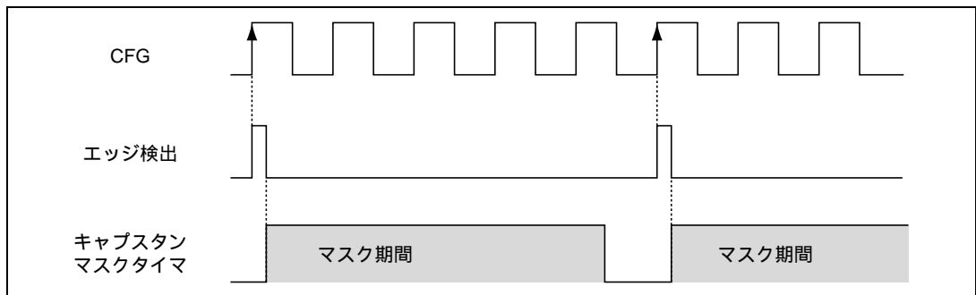
図 26.69 CFG マスクタイマの動作例 (キャプスタンモータ正常動作時)
