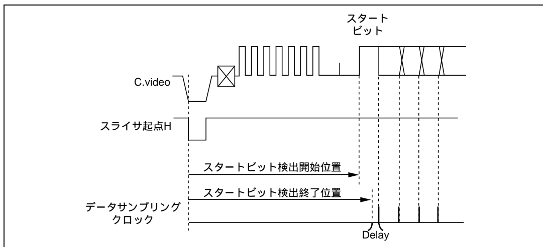
図 28.6 スタートビット未検出時のデータサンプリングクロック
