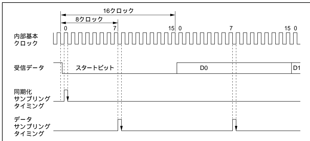
図 22.23 調歩同期式モードの受信データサンプリングタイミング
