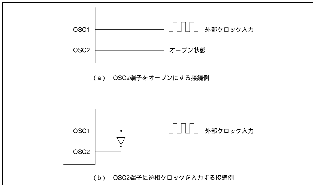
図 9.5 外部クロックの接続例
