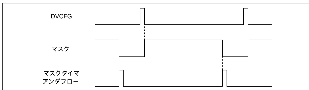
図 26.67 マスク信号
