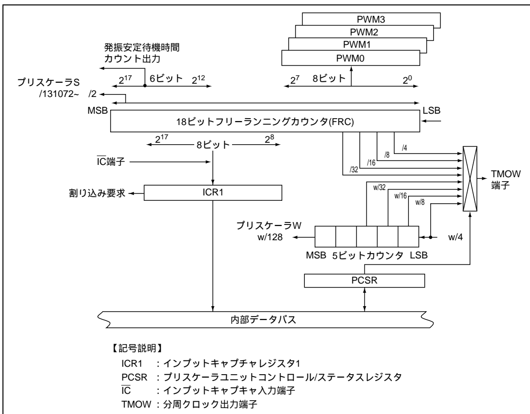
図 21.1 プリスケラユニットのブロック図
