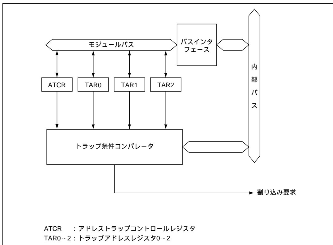
図 25.1 ATC のブロック図
