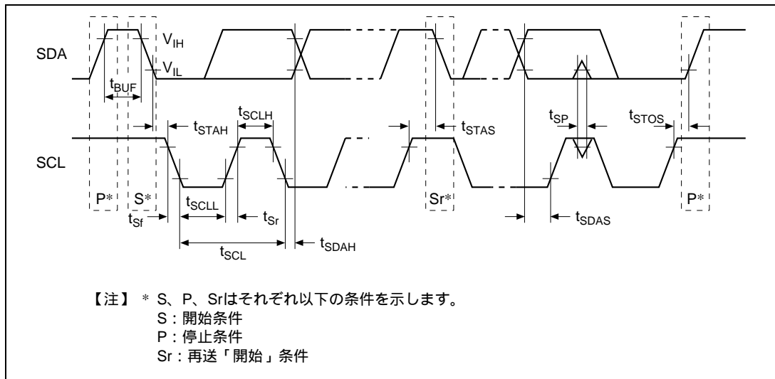
図 31.16 I 2 C バスインタフェース入出力タイミング
