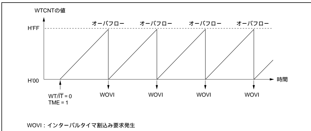
図 17.4 インターバルタイマモード時の動作
