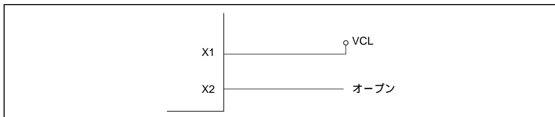
図 9.10 サブクロックを使用しない場合の端子処理
