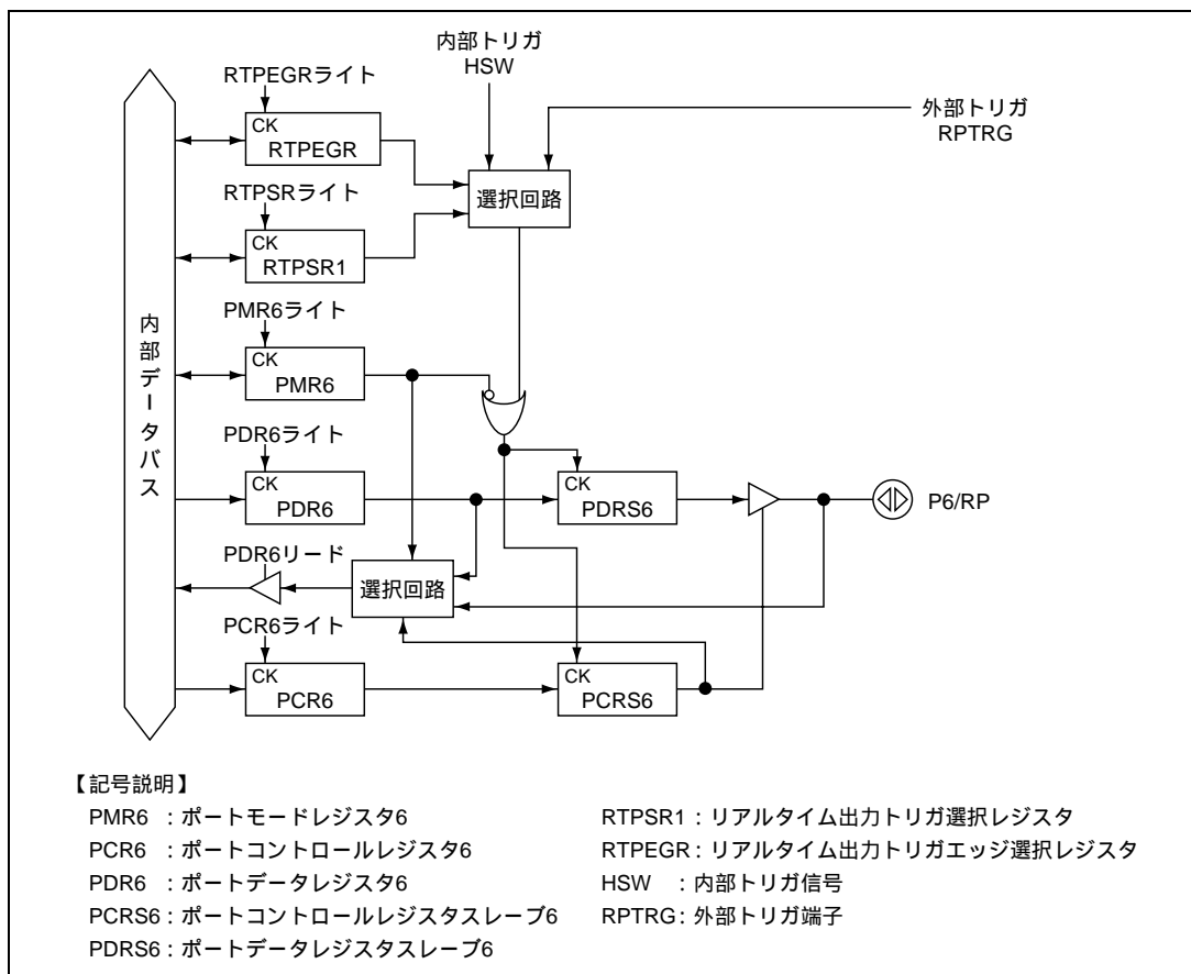
図 10.2 ポート 6 の機能ブロック図
