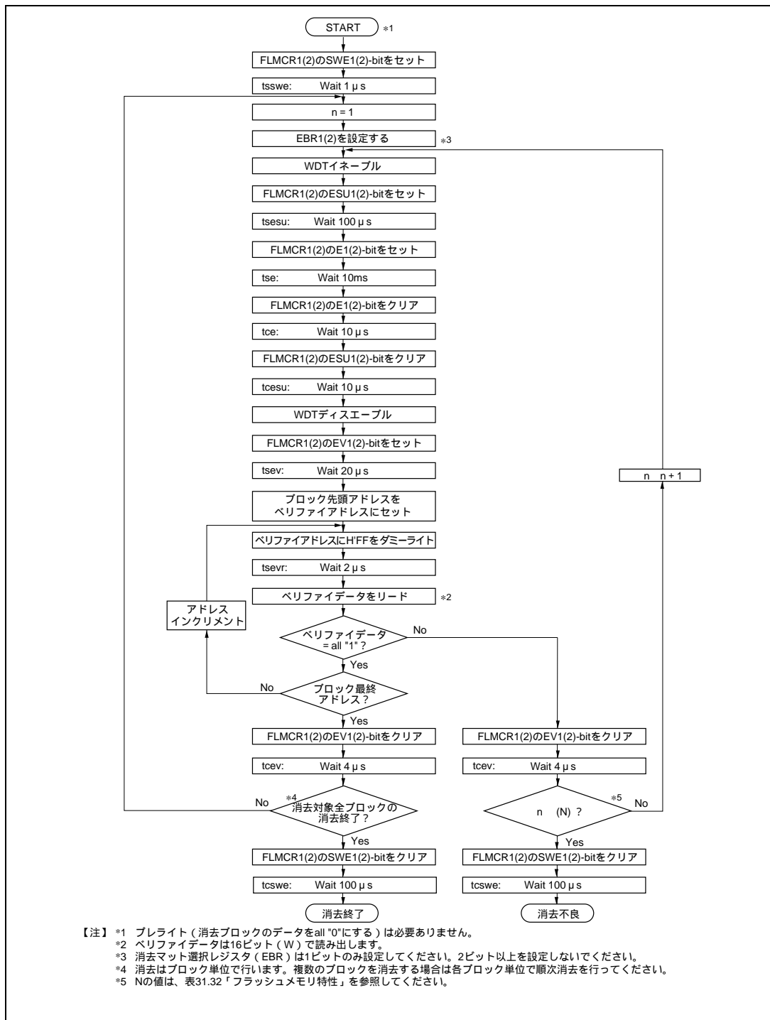
図 7.13 イレース/イレースベリファイフロー
