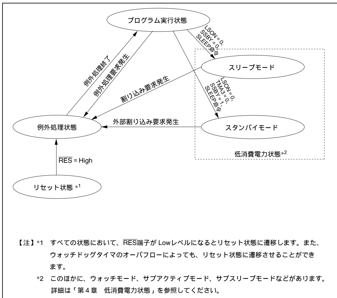
図 2.16 状態遷移図
