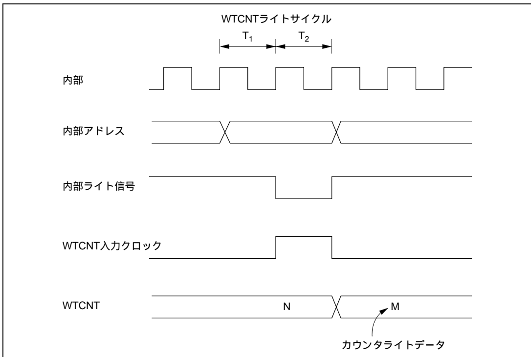
図 17.6 WTCNT のライトとカウントアップの競合
