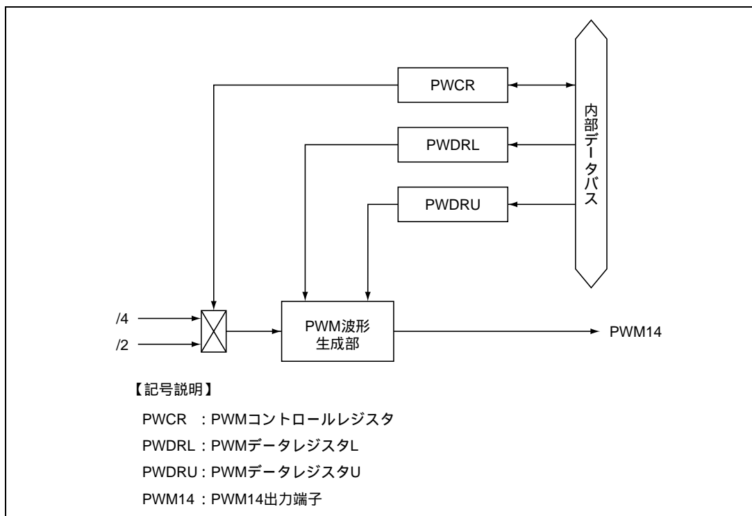
図 20.1 14ビットPWMのブロック図
