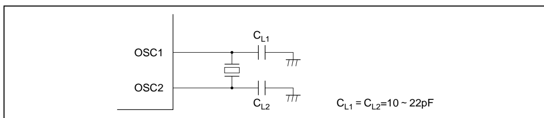
図 9.2 水晶発振子の接続例
