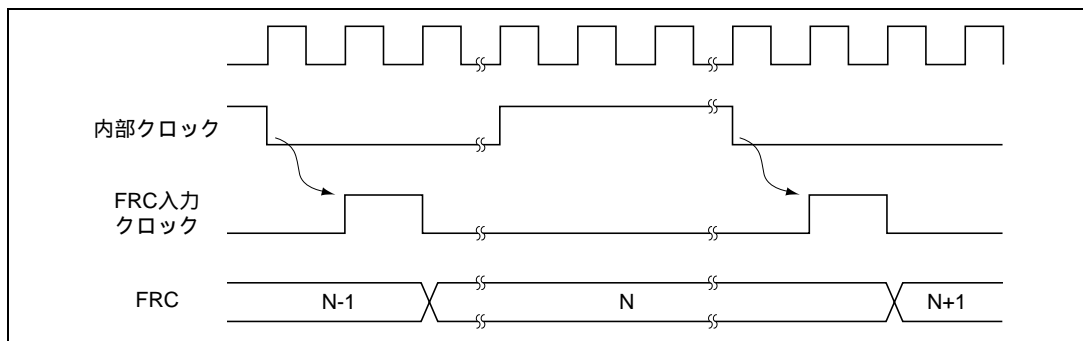
図 16.3 内部クロック動作時のカウントタイミング
