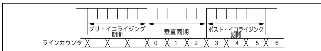
図 29.10 垂直方向の表示開始位置の起点
