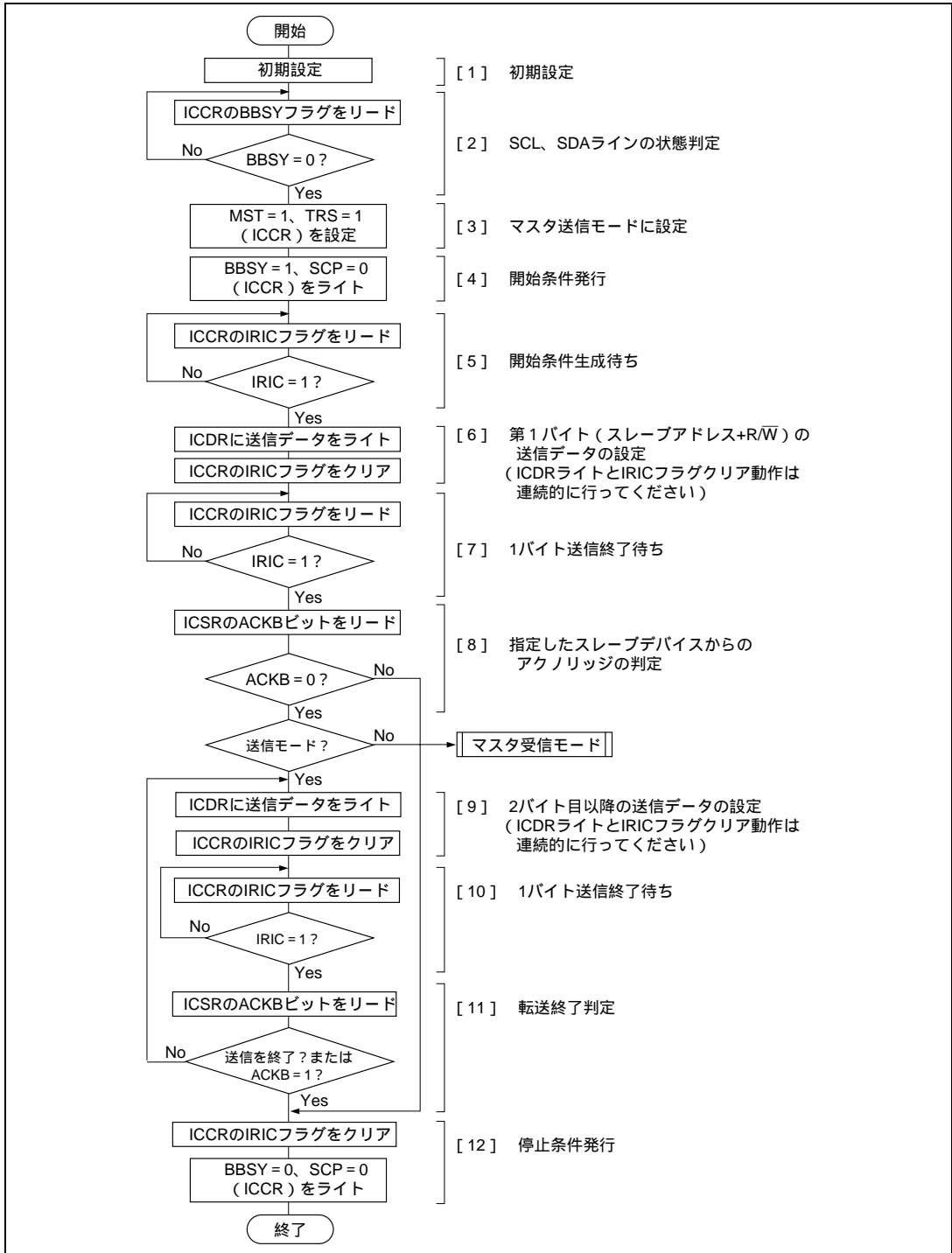
図 23.14 マスタ送信モードのフローチャート例
