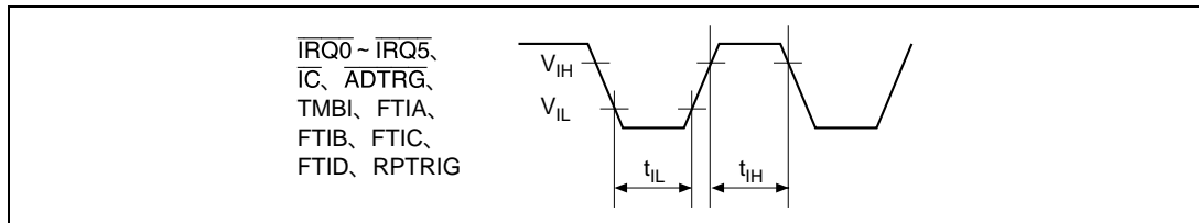
図 31.4 入力タイミング
