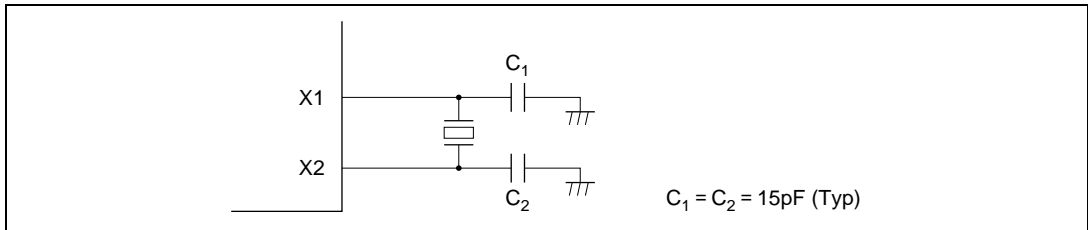
図 9.8 32.768kHz 水晶発振子の接続例
