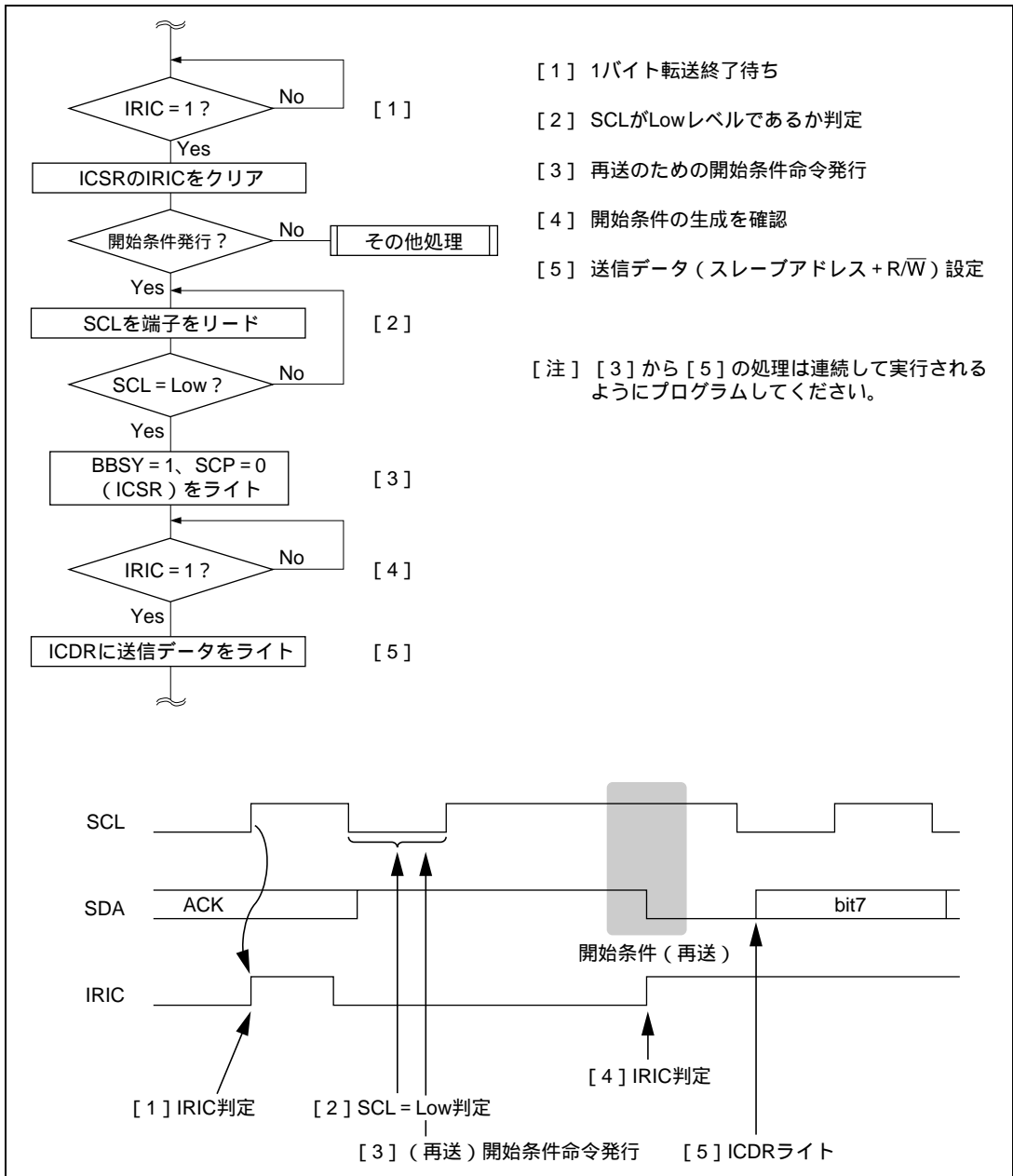
図 23.19 再送のための開始条件命令発行フローチャートおよびタイミング
