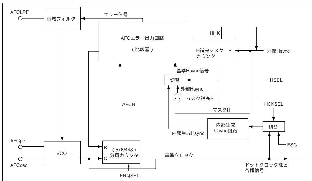
図 27.22 AFC 回路のシステム構成
