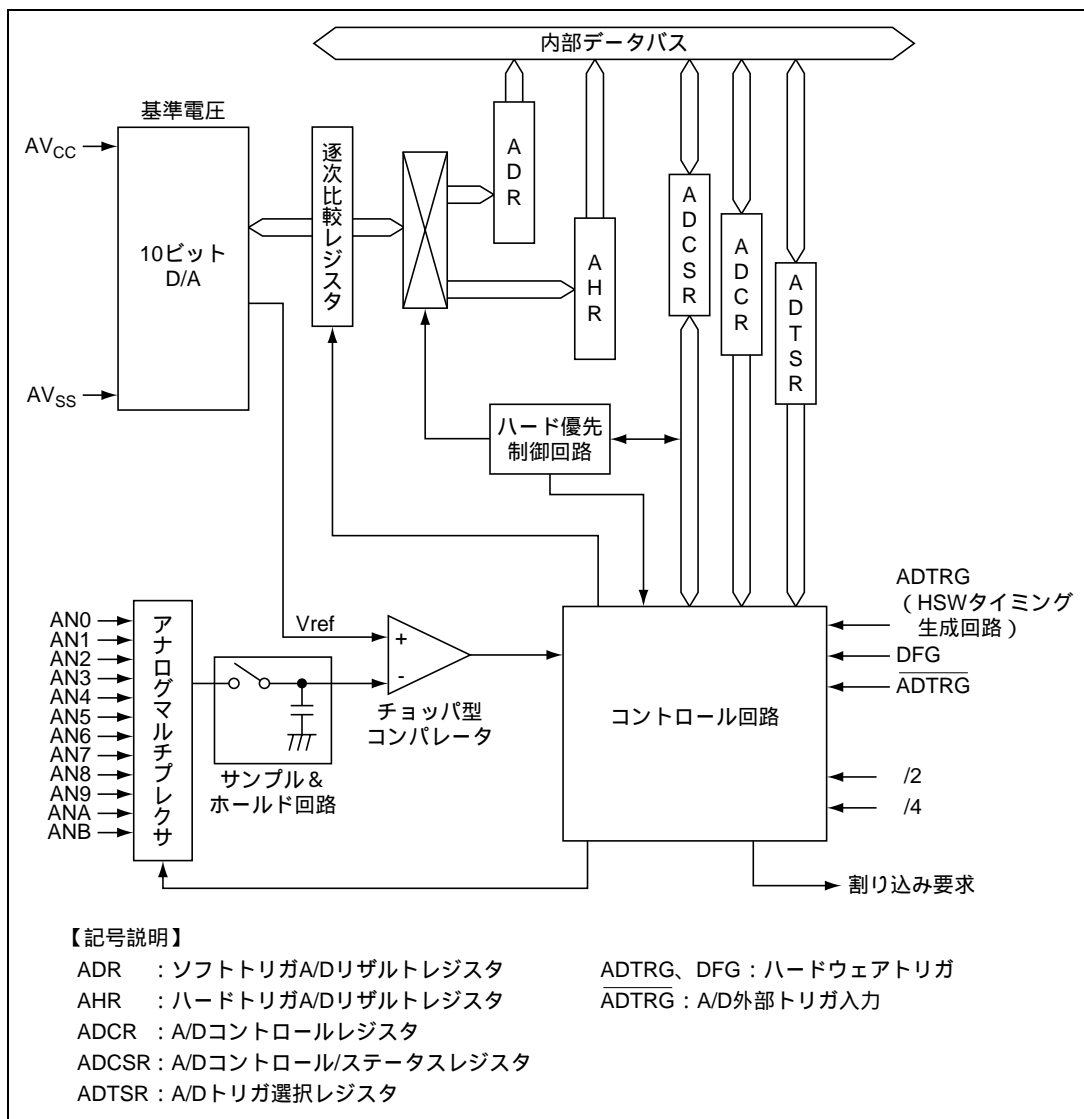
図 24.1 A/D 変換器ブロック図
