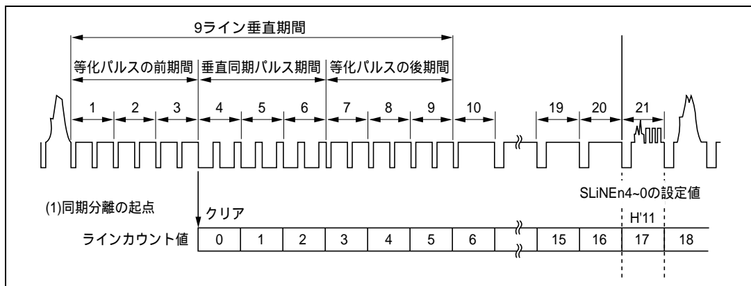
図 28.4 ラインカウント値
