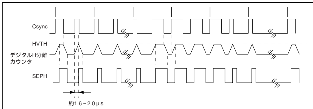
図 27.3 等価パルス検出時の HVTH 設定と SEPH 生成のタイミング
