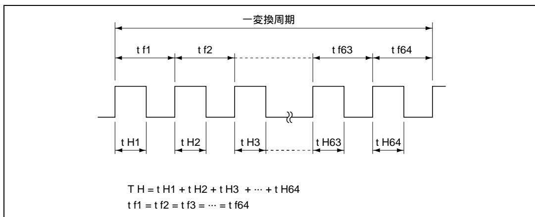
図 20.2 14ビットPWM出力波形
