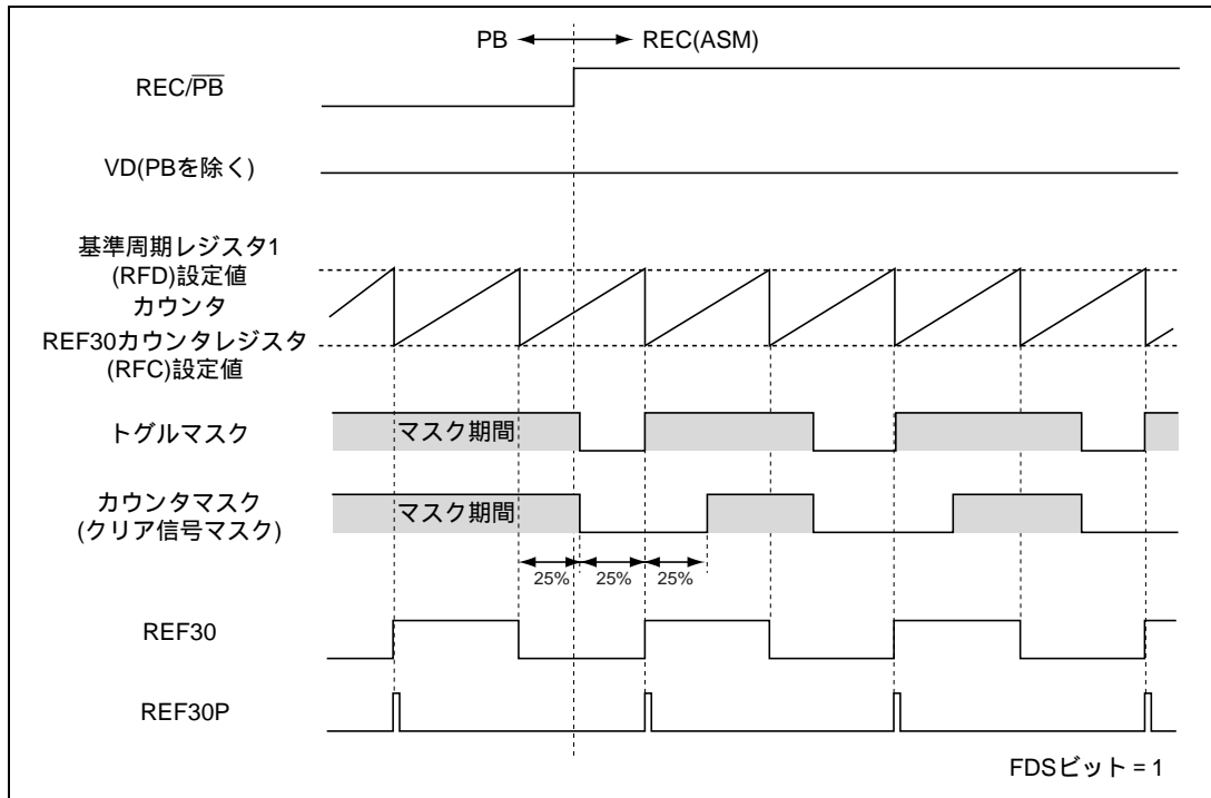
図 26.19 RFD ビット = 1 の時、PB REC 切り替え時の基準信号の生成 (VD 信号未検出時) (2)
