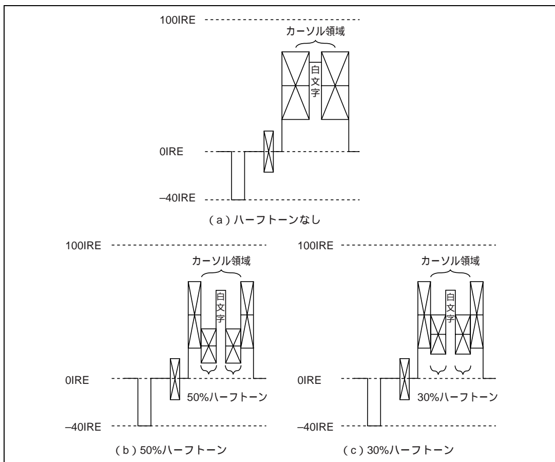
図 29.9 ハーフトーン階調 (例) (C. Video)
