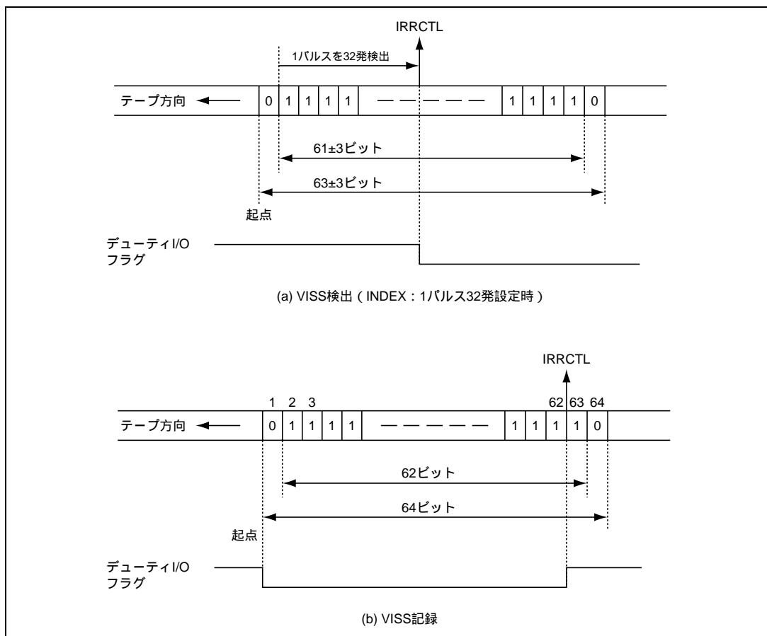
図 26.57 VISS ビット列とデューティ I/O フラグ
