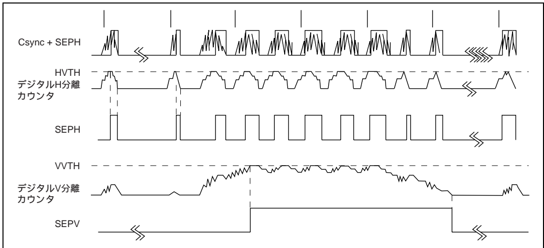
図 27.11 デジタル LPFON 時の VVTH 設定と SEPV 生成のタイミング
