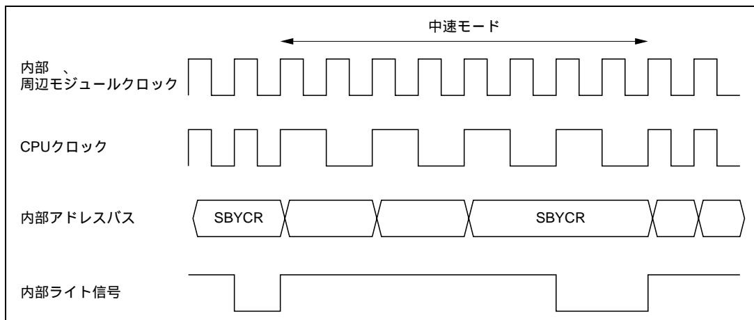
図 4.2 中速モードの遷移・解除タイミング
