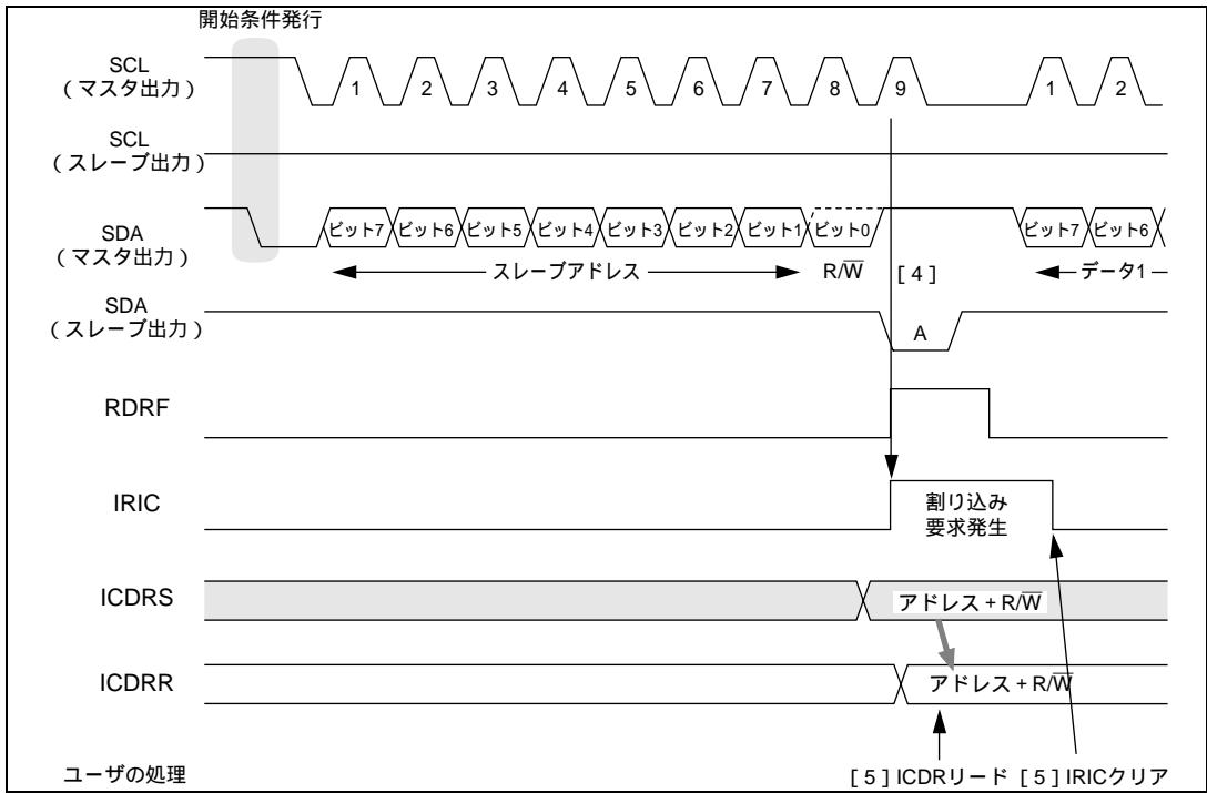
図 23.9 スレーブ受信モード動作タイミング例 1 (MLS = ACKB = 0 のとき)
