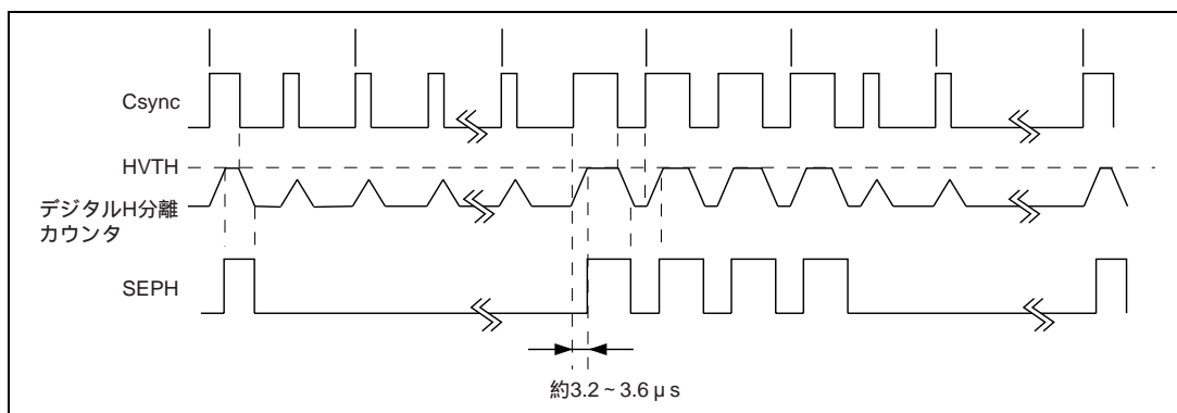
図 27.4 等価パルス未検出時の HVTH 設定と SEPH 生成のタイミング
