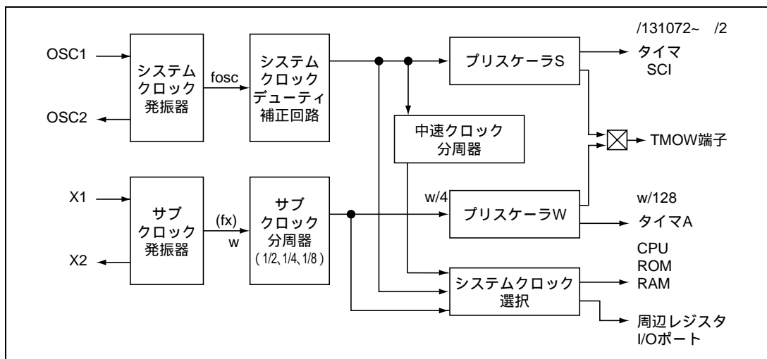
図 21.2 クロック供給
