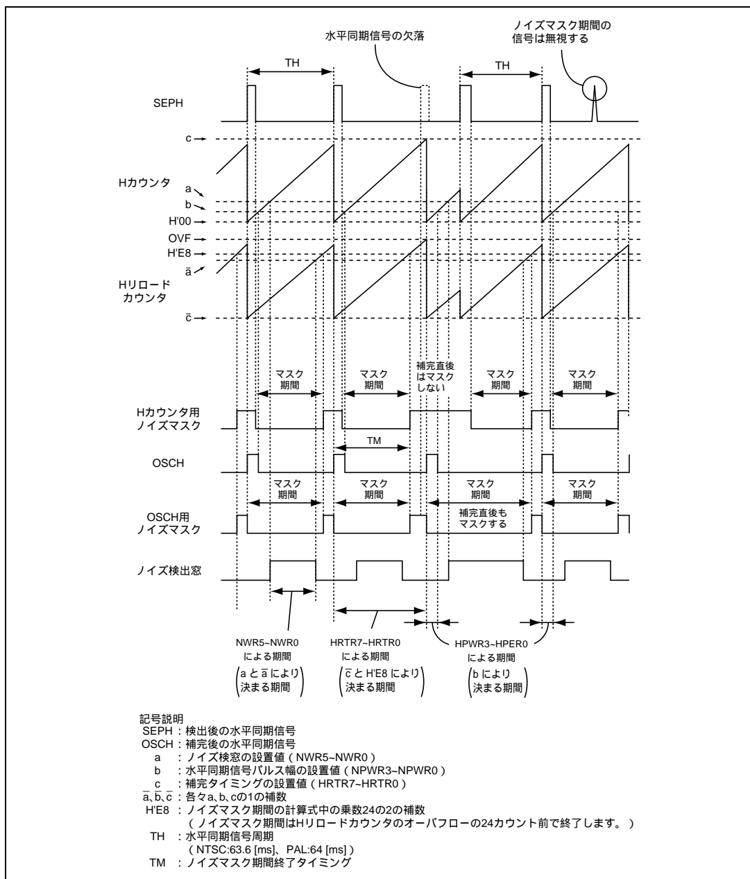
図 26.75 HRTR、HPWR、NWR の設定期間
