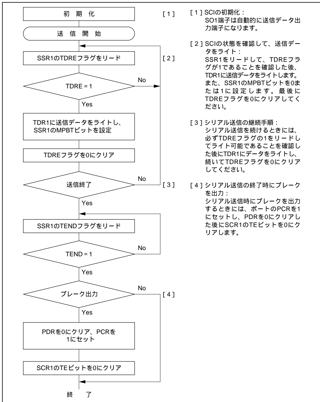
図 22.11 マルチプロセッサシリアル送信のフローチャートの例
