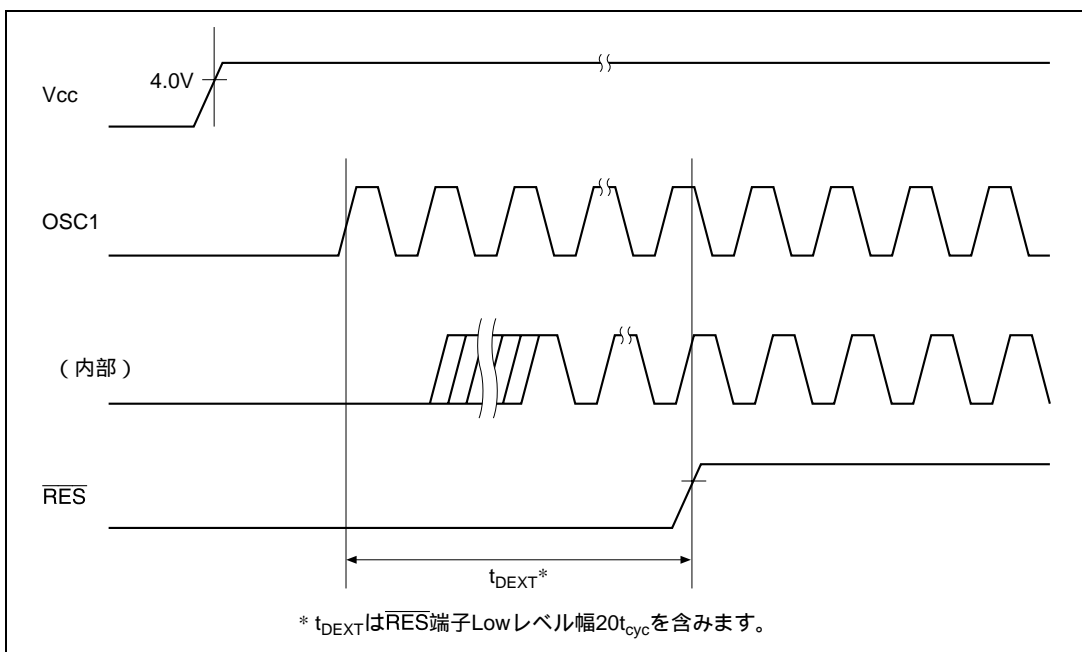
図 31.2 外部クロック安定遅延時間タイミング
