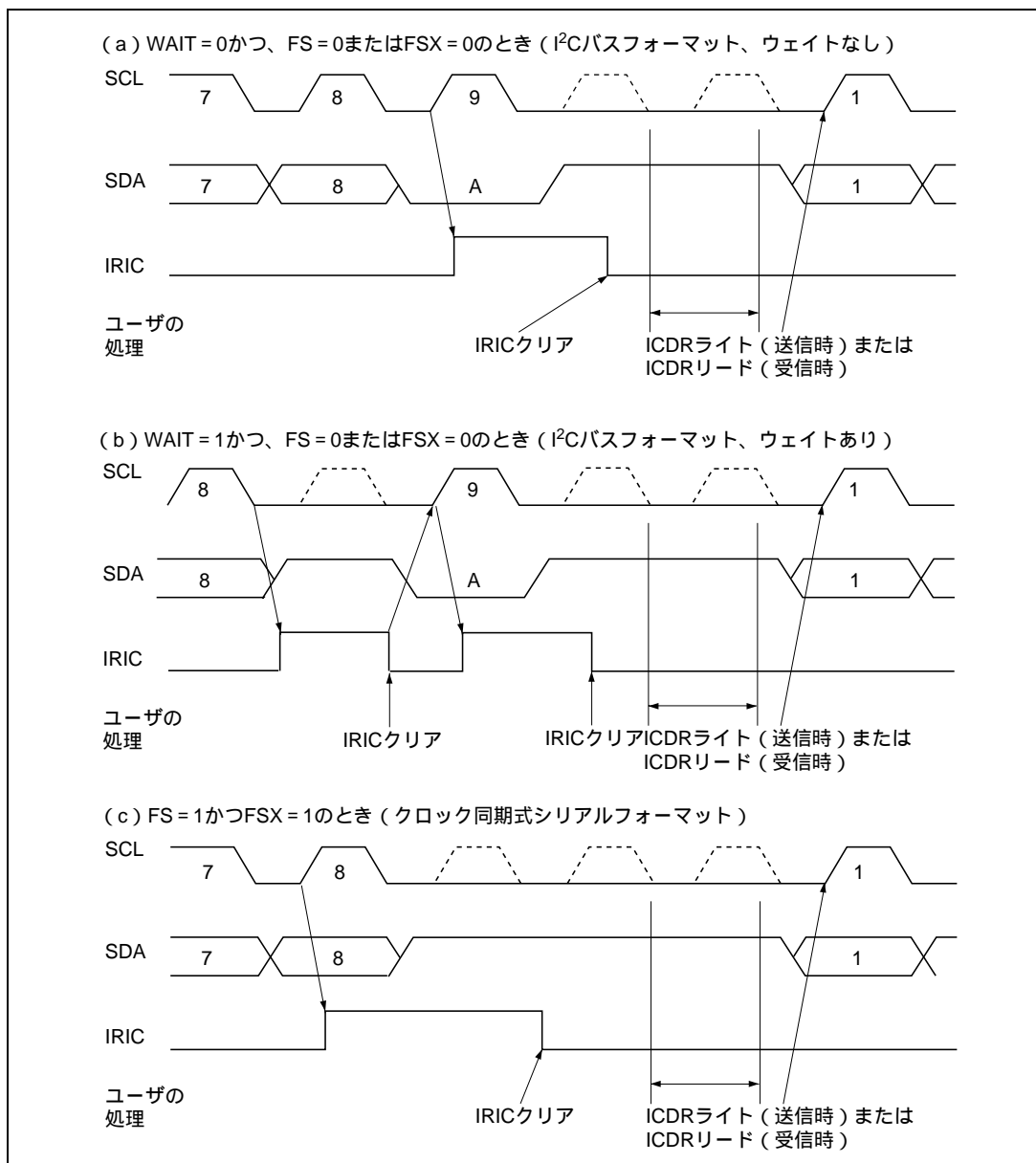
図 23.12 IRIC セットタイミングと SCL 制御
