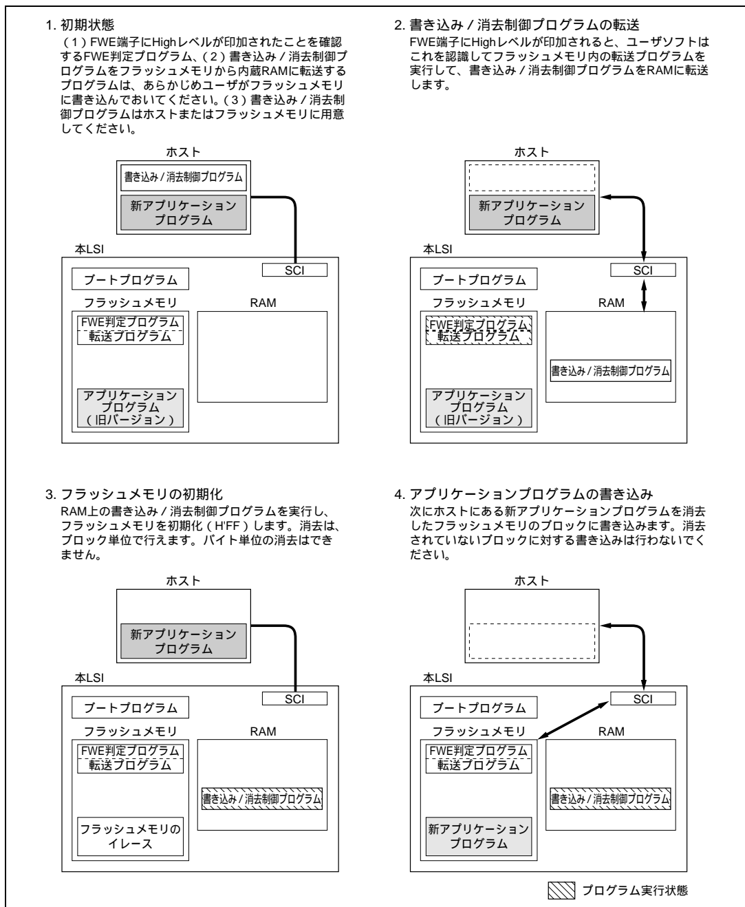
図 7.5 ユーザプログラムモード (例)
