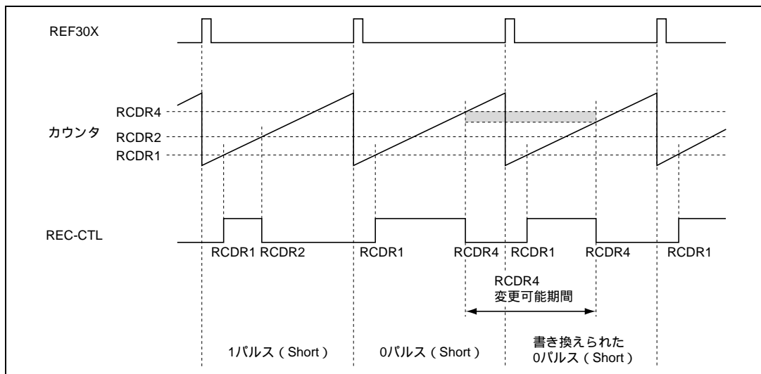
図 26.61 RCDR の変更タイミング例 (RCDR4)
