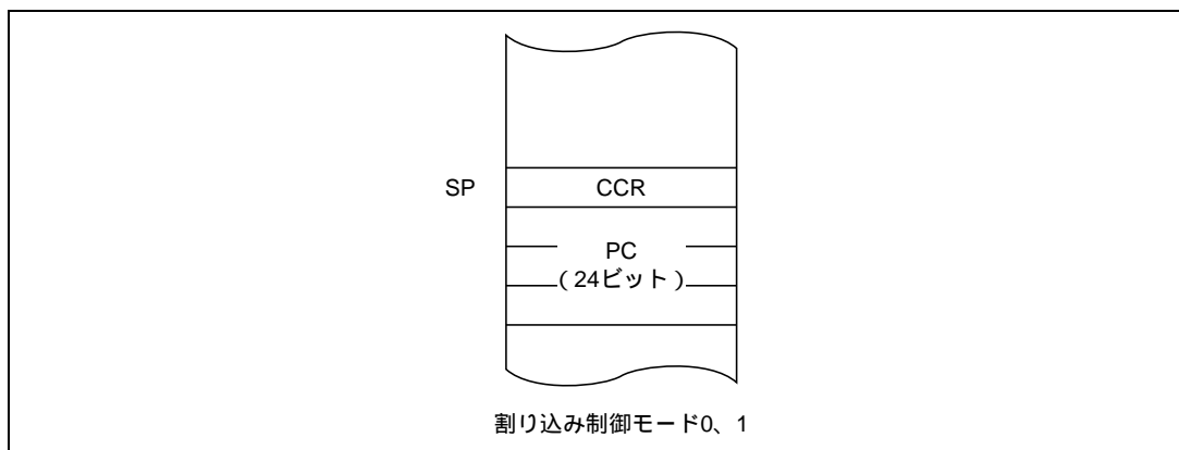
図 5.5 例外処理終了後のスタックの状態（アドバンスモード）
