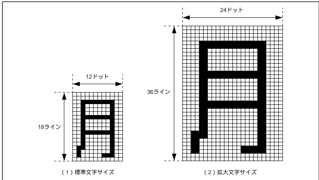
図 29.3 拡大文字
