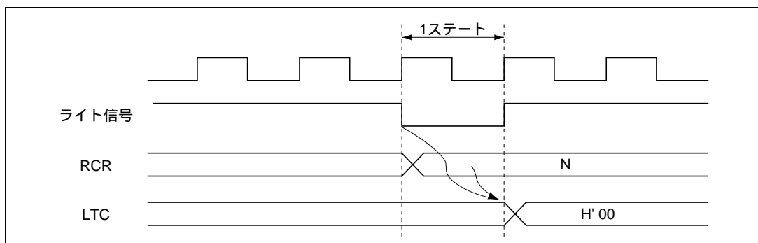
図 14.2 RCR ライト、LTC クリアタイミング
