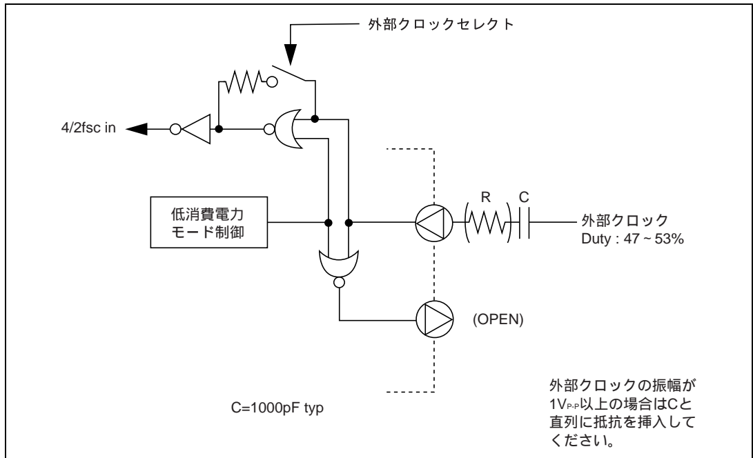
図 29.22 4/2fsc 外部クロックの入力例
