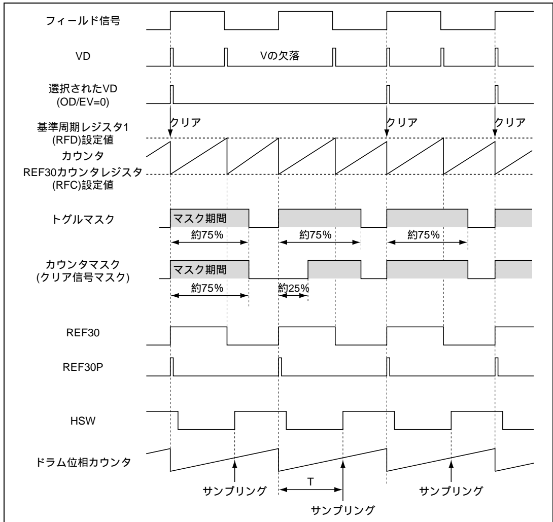
図 26.10 記録時の基準信号の生成 (Vの欠落)
