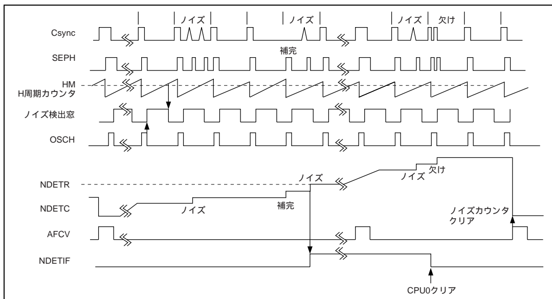
図 27.15 ノイズ検出窓設定とノイズカウンタのタイミング
