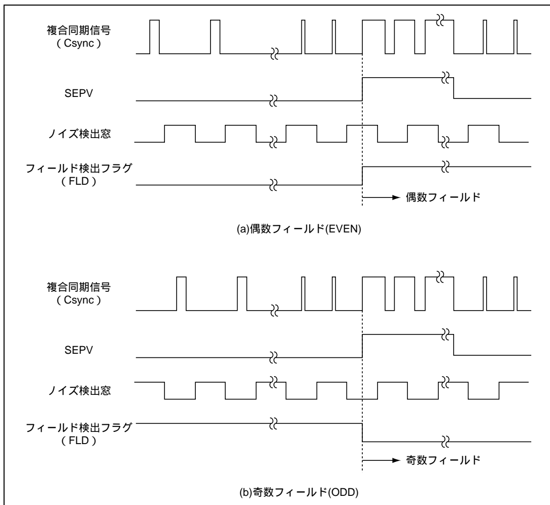
図 26.74 フィールド検出
