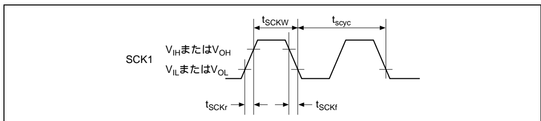
図 31.21 SCK1 クロックタイミング
