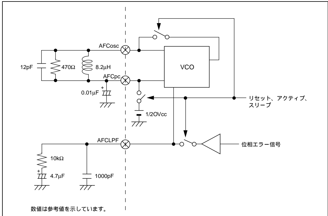
図 27.23 基準クロック周波数 (576 × fh) を選択した場合の回路例
