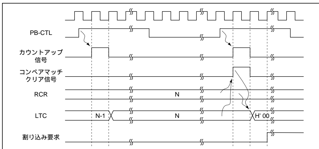
図 14.3 コンペアマッチクリアタイミング (PB-CTL の立ち上がりエッジ選択時)
