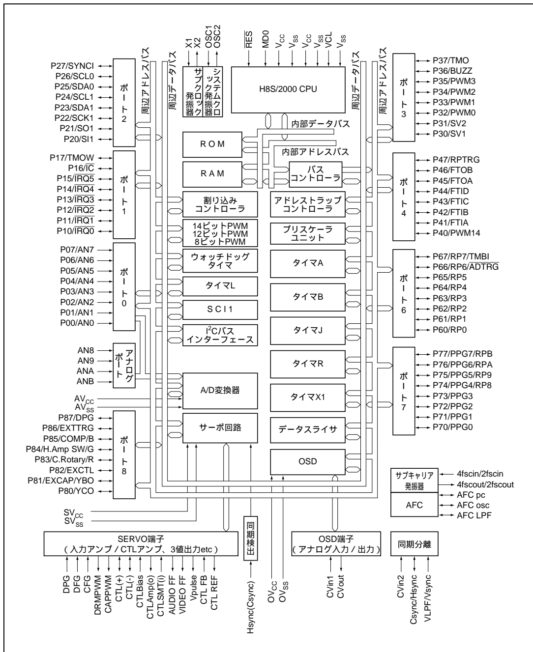
図 1.1 H8S/2199R グループの内部ブロック図 (H8S/2197S、H8S/2196S を除く)
