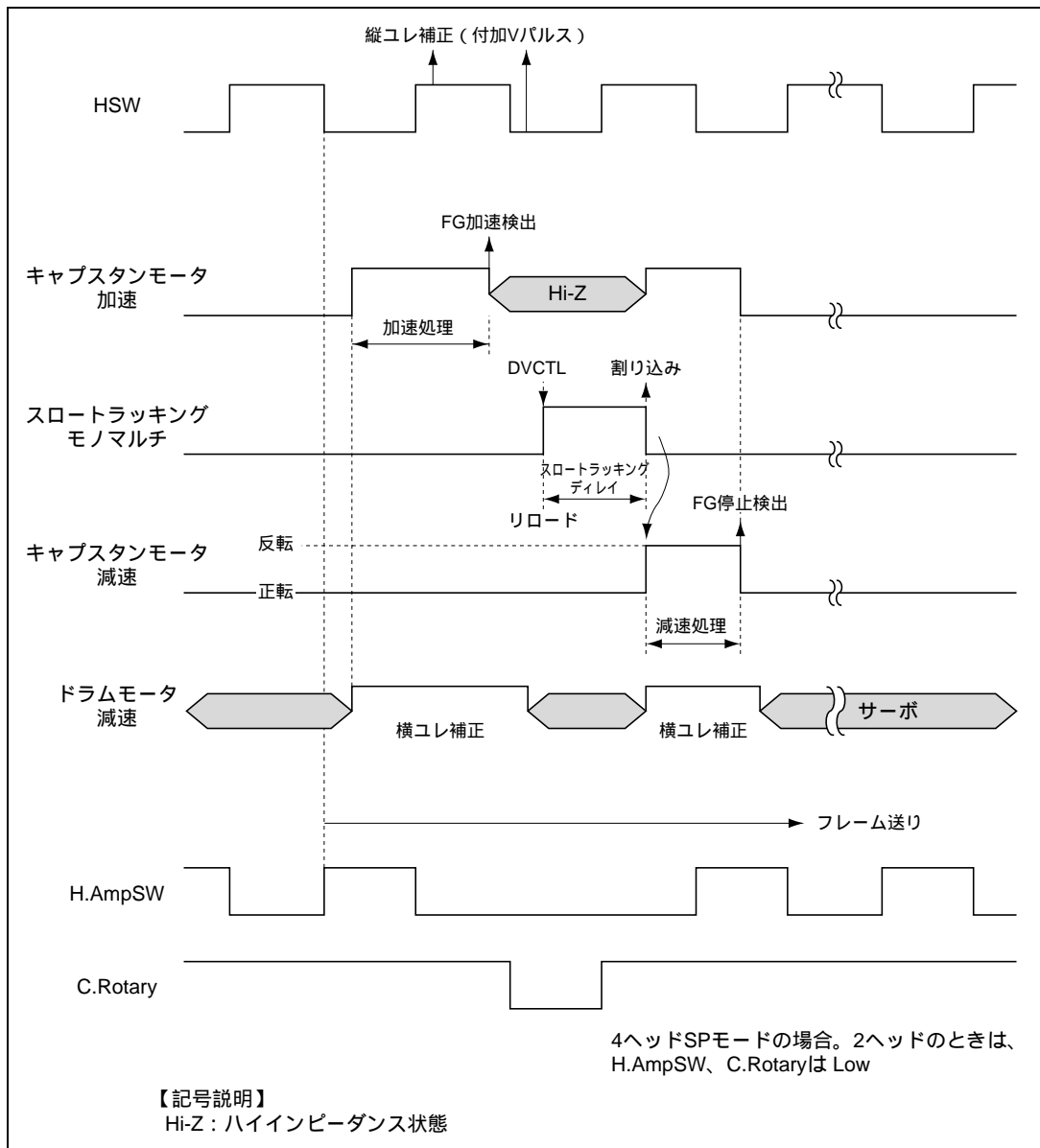
図 15.2 スロー再生時の時系列動作例
