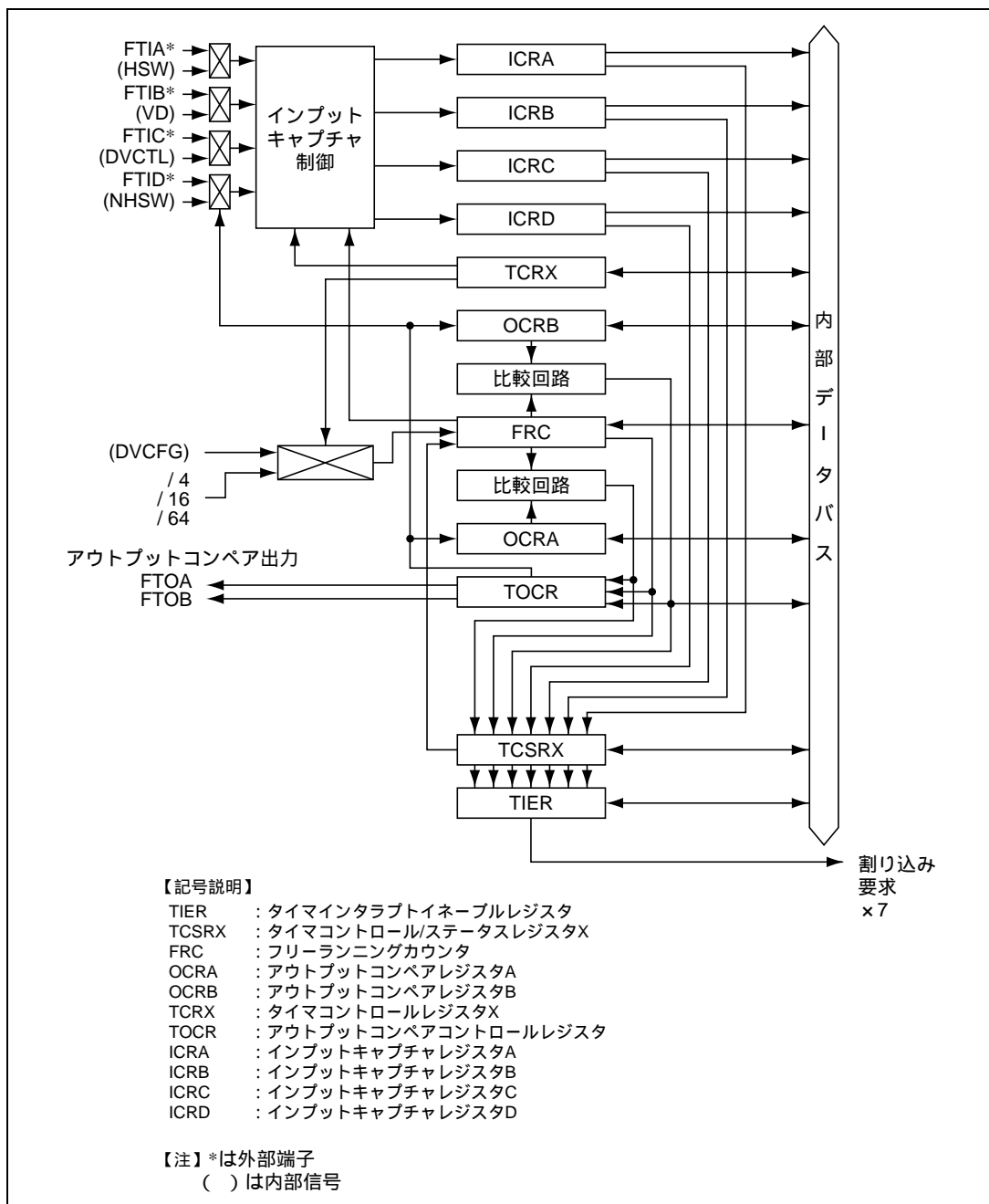
図 16.1 タイマ X1 ブロック図
