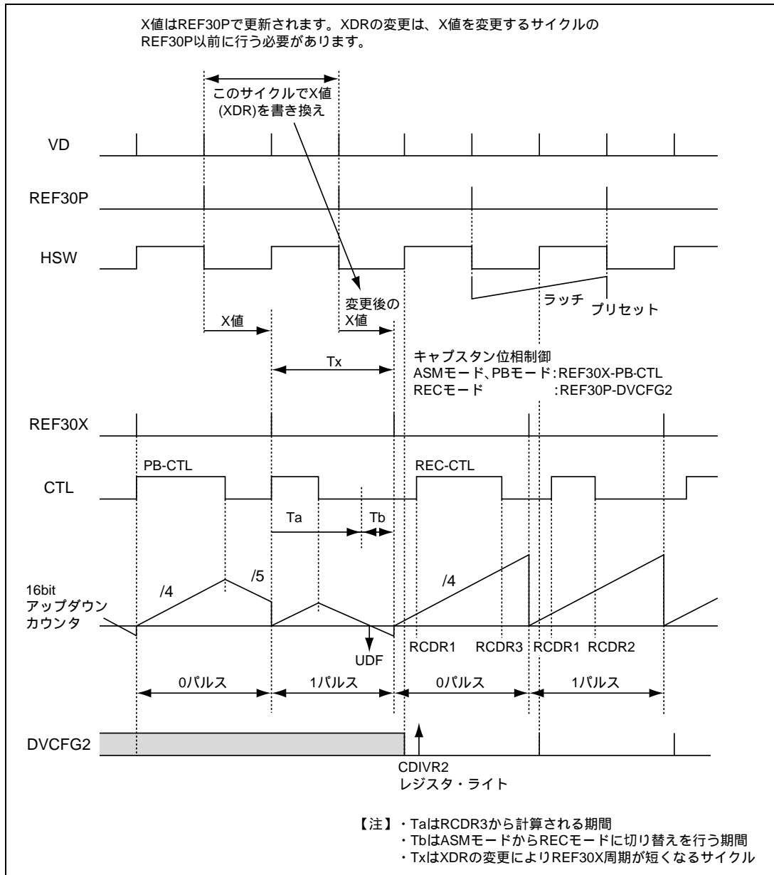
図 26.50 CTLM 切り替えタイミング例 (REC時、REF30P と DVCFG2 で位相制御する場合)
