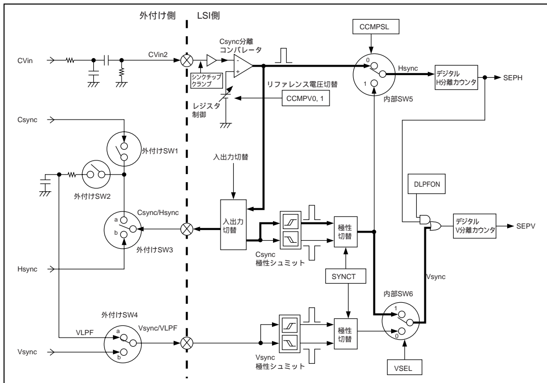
図 27.18 Cvin2 入力で Csync シュミットを使用した場合の分離入力
