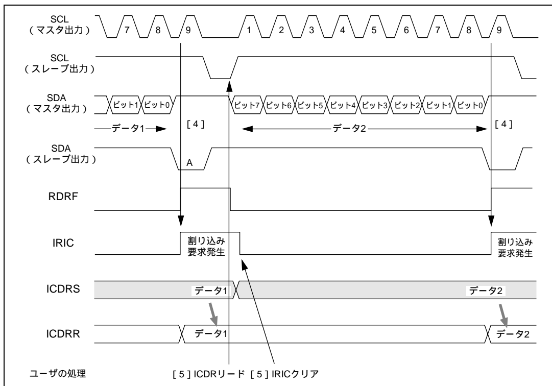
図 23.10 スレーブ受信モード動作タイミング例 2 (MLS = ACKB = 0 のとき)
