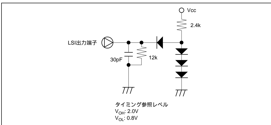
図 31.23 出力負荷条件
