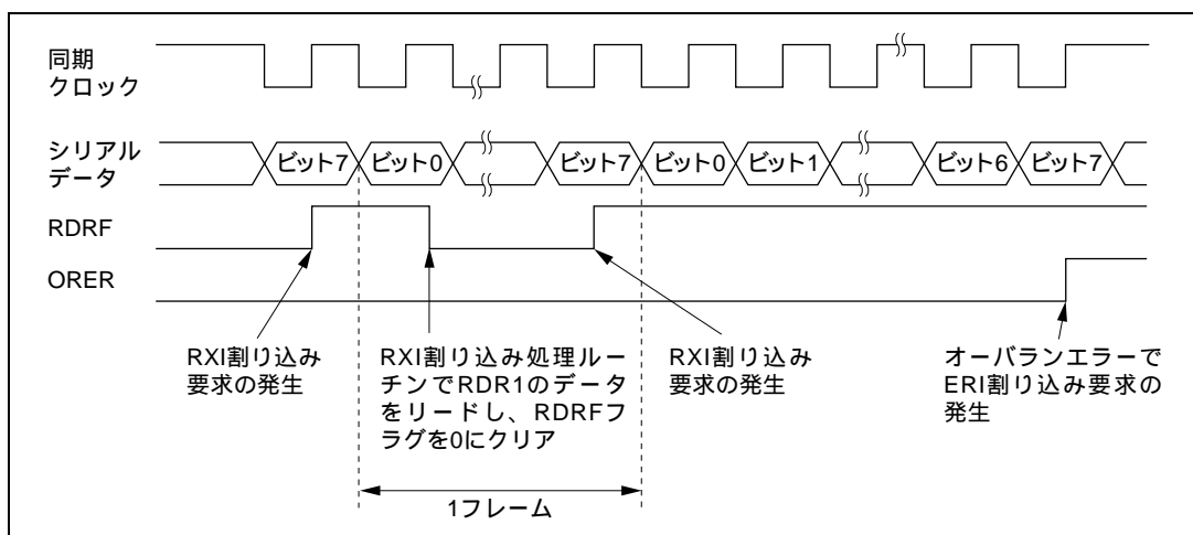
図 22.21 SCI の受信時の動作例
