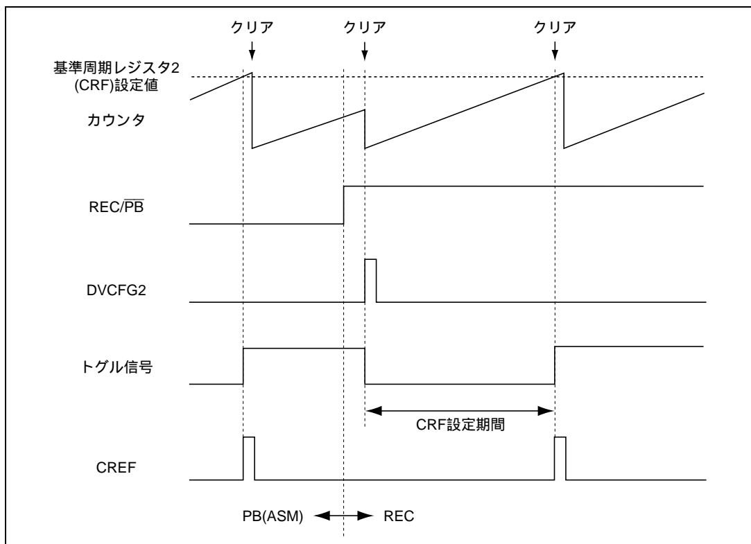
図 26.15 PB REC 時の CREF 信号 (CRD ビット = 1 の時)
