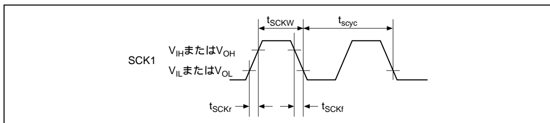
図 31.5 SCK1 クロックタイミング
