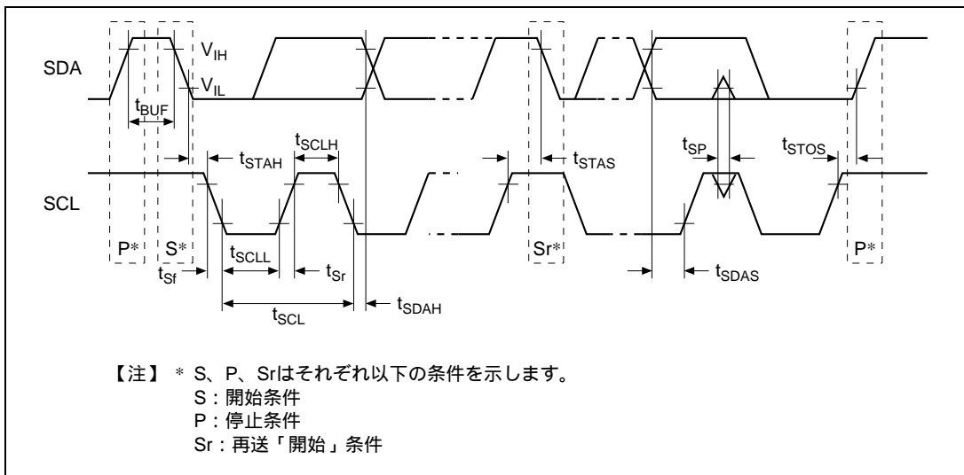
図 31.8 I 2 C バスインタフェース入出力タイミング
