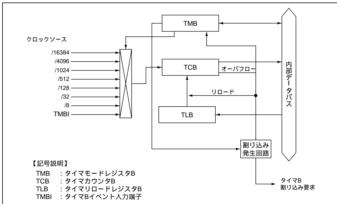
図 12.1 タイマ B ブロック図
