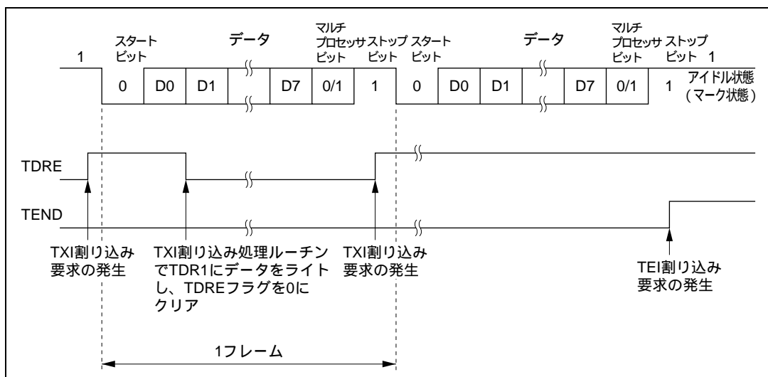
図 22.12 SCI の送信時の動作例 (8ビットデータ/マルチプロセッサビットあり/1ストップビットの例)
