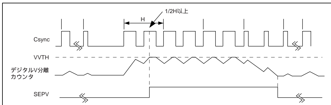
図 27.10 VVTH 設定と SEPV 生成のタイミング
