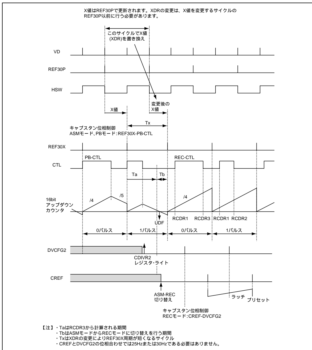
図 26.51 CTLM 切り替えタイミング例 (REC時、CREFとDVCFG2で位相制御する場合)
