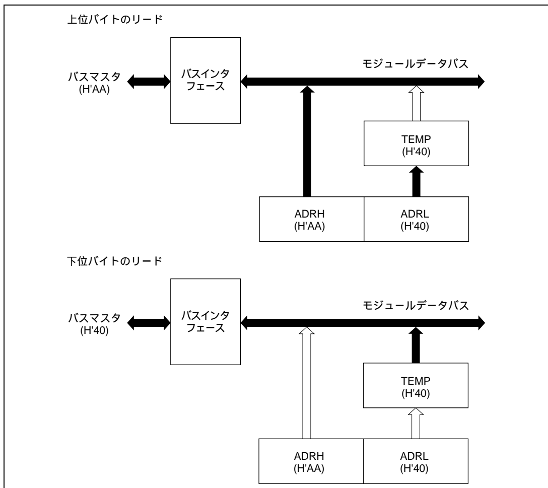
図 24.3 ADR のアクセス動作 (H'AA40 リード時)
