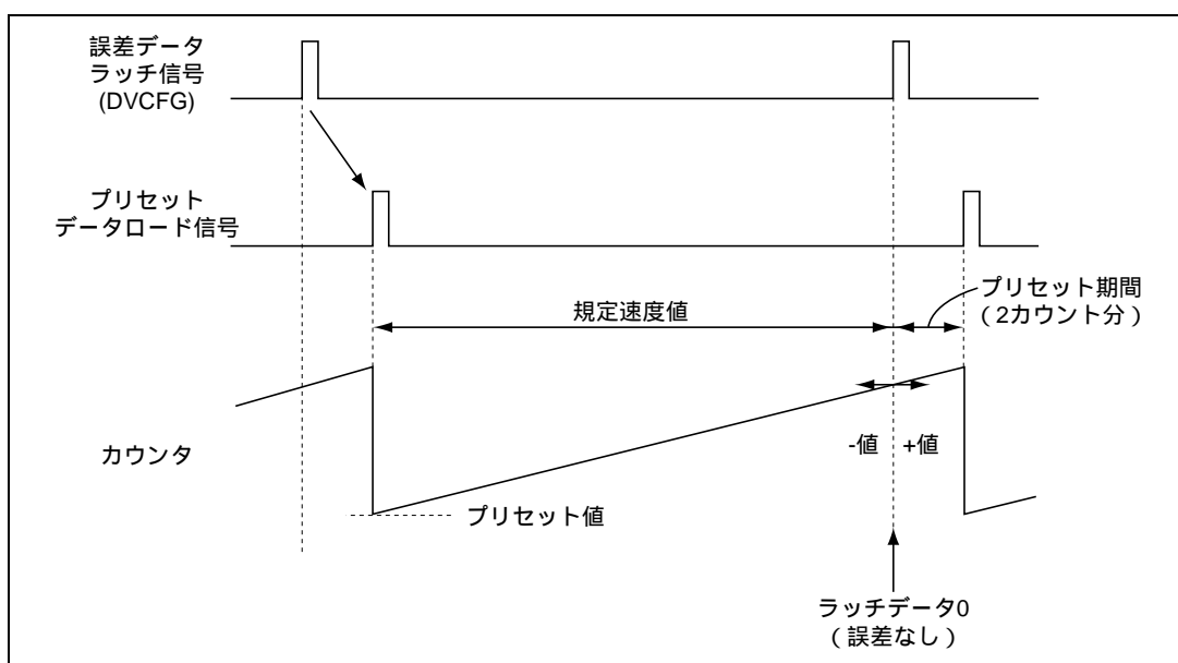
図 26.33 キャプスタン速度誤差検出の動作例
