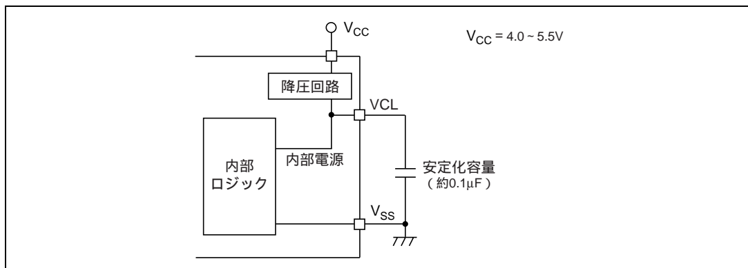
図 30.1 内部電源降圧回路を使用する場合の電源接続図
