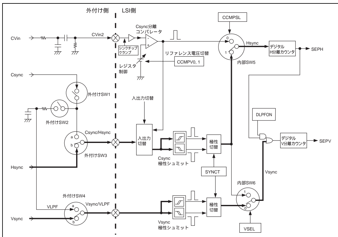
図 27.21 Hsync/Vsync 入力した場合の分離入力
