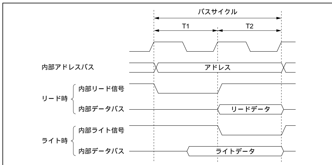
図 2.19 内蔵周辺モジュールアクセスサイクル
