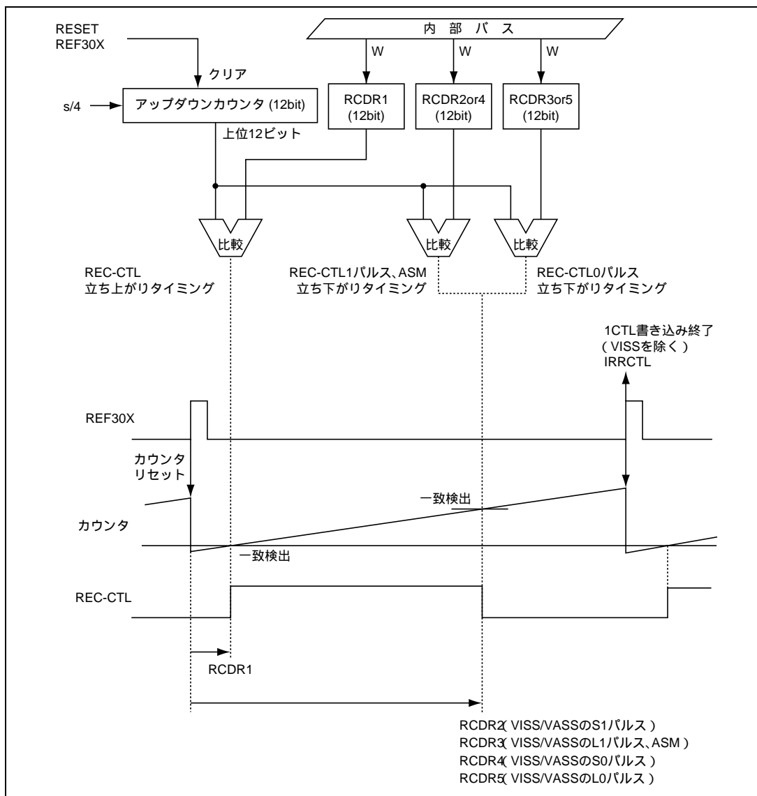
図 26.60 REC-CTL 信号生成タイミング
