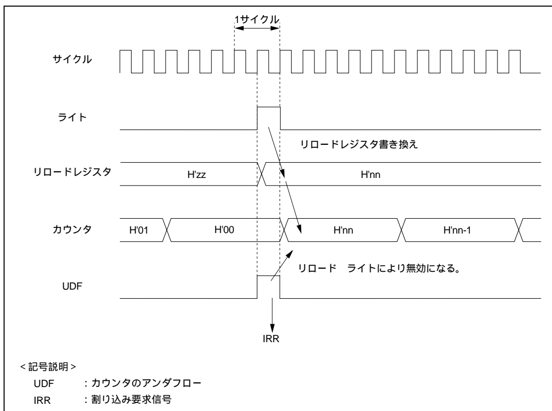
図 14.7 リロードタイマのアンダフローとリロードレジスタ書き換えの競合
