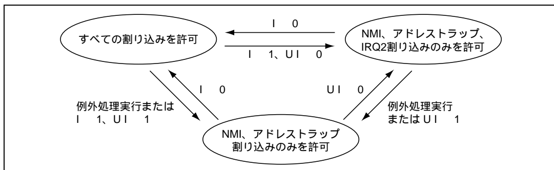
図 6.6 割り込み制御モード 1 の状態遷移例
