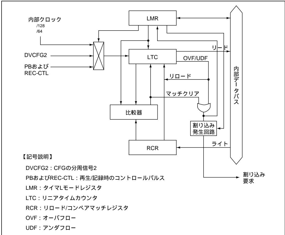
図 14.1 タイマ L ブロック図
