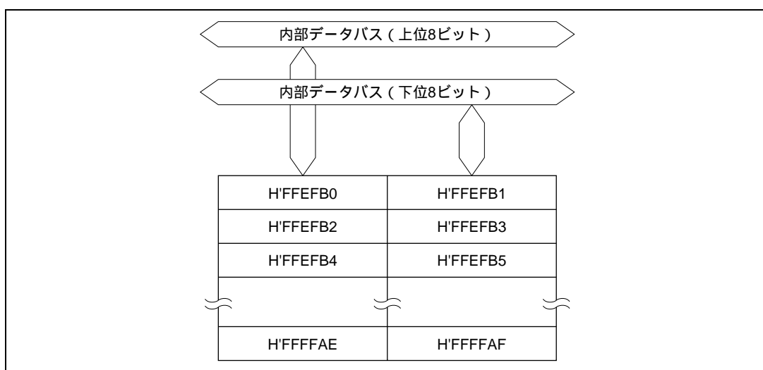
図 8.1 RAM のブロック図 (H8S/2199R の場合)
