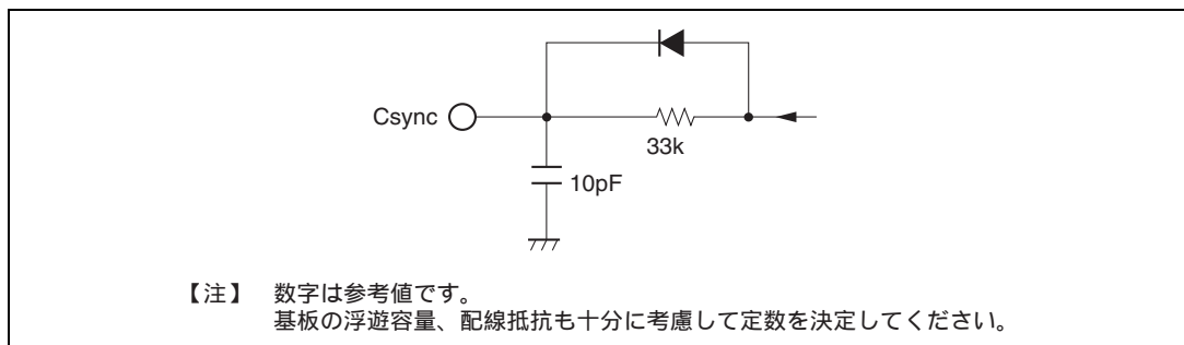
図 E.6 同期信号検出回路部の外部回路例
