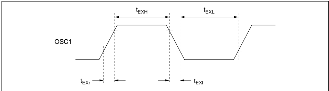
図 9.6 外部クロック入力タイミング
