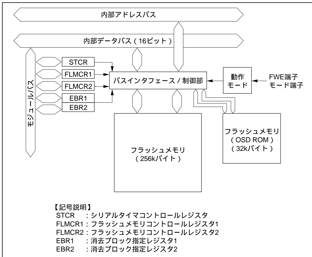
図 7.2 フラッシュメモリのブロック図 (H8/2199R のみ)
