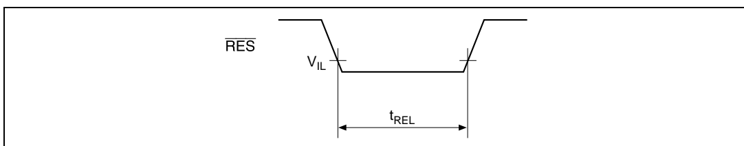
図 31.3 リセット入力タイミング
