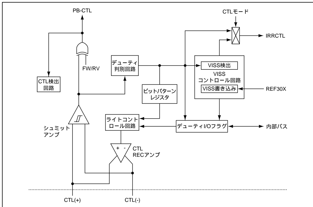
図 26.47 CTL 回路のブロック図
