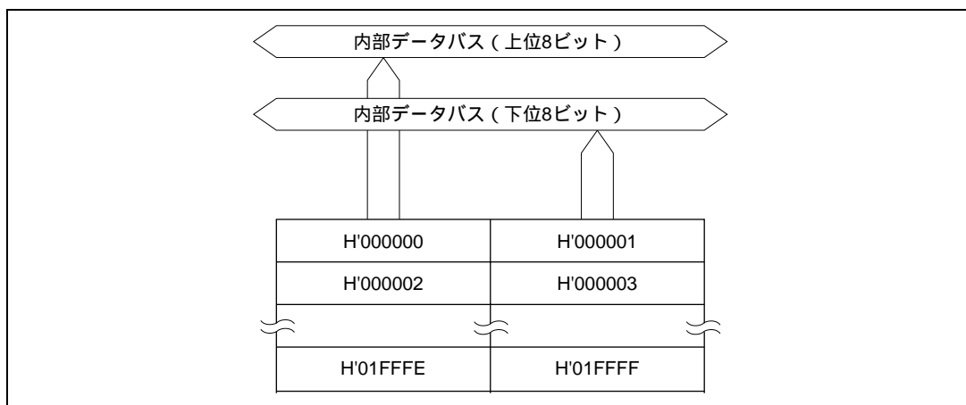
図 7.1 ROM のブロック図 (H8S/2199R の例)
