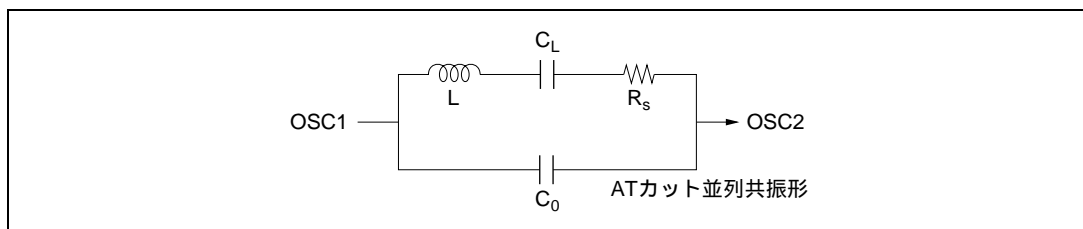
図 9.3 水晶発振子の等価回路
