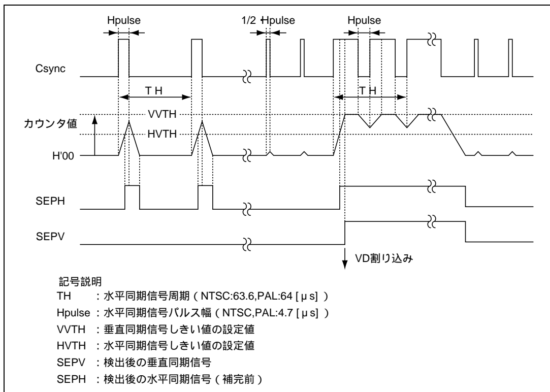
図 26.73 しきい値と分離された同期信号
