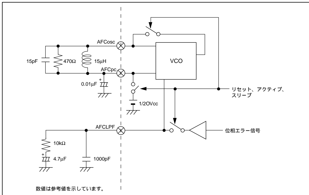
図 27.24 基準クロック周波数 448 \times f_h を選択した場合の回路例
