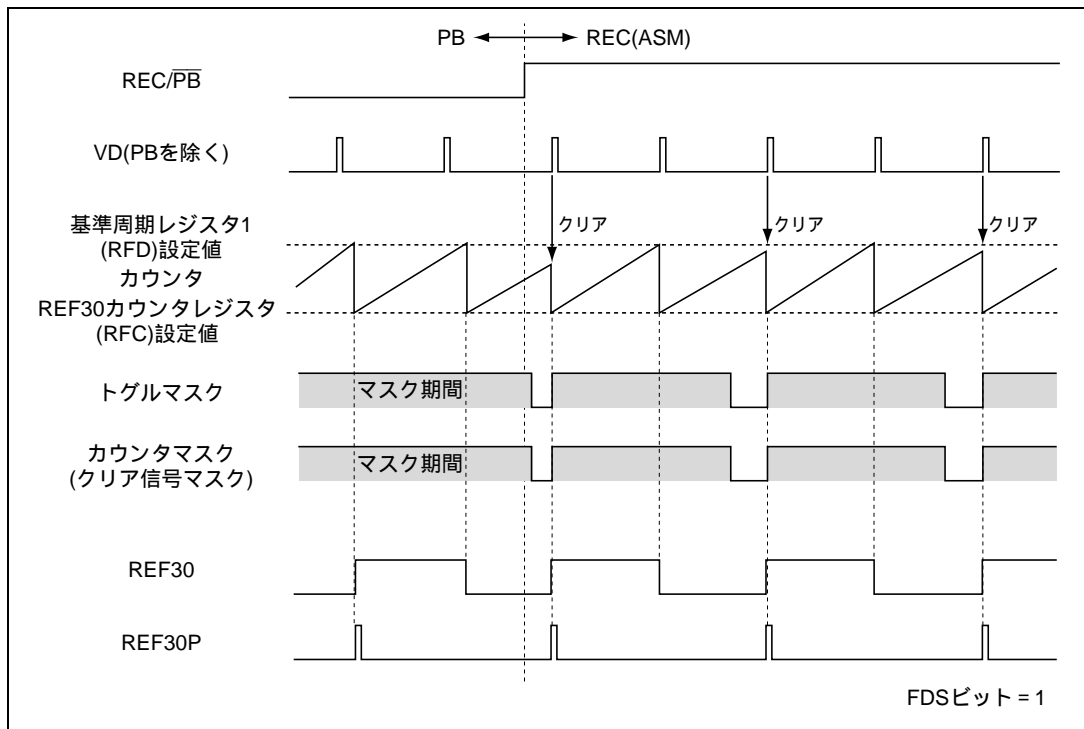
図 26.18 RFD ビット = 1 の時、PB REC 切り替え時の基準信号の生成 (1)
