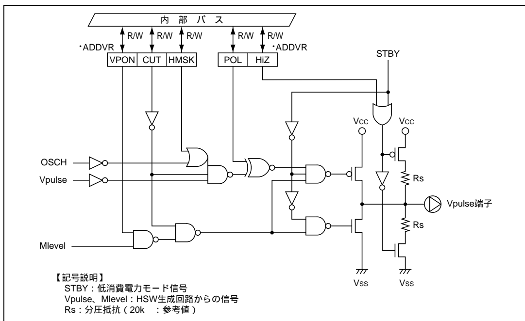
図 26.44 付加Vパルス端子
