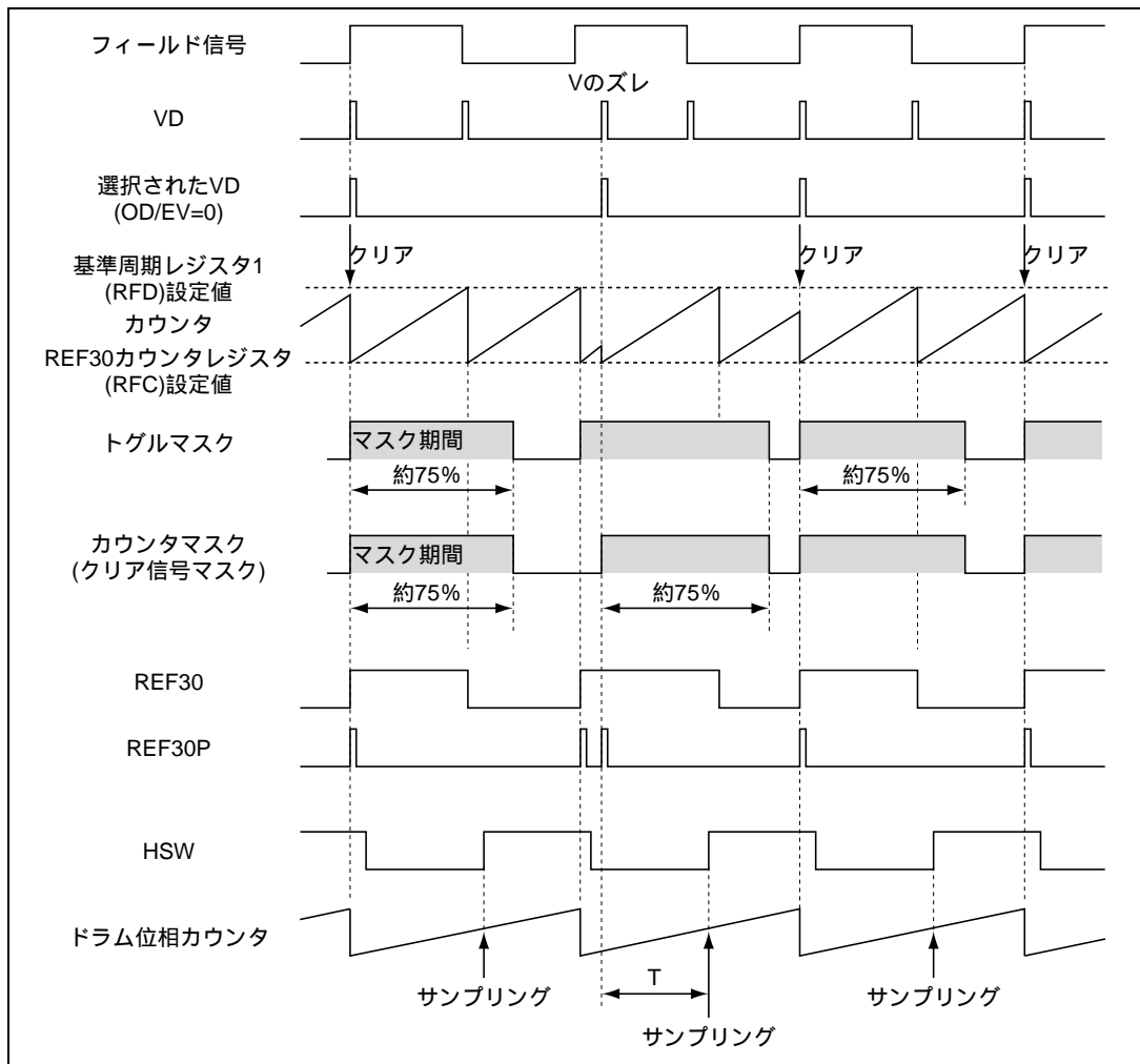
図 26.11 記録時の基準信号の生成 (Vのズレ)
