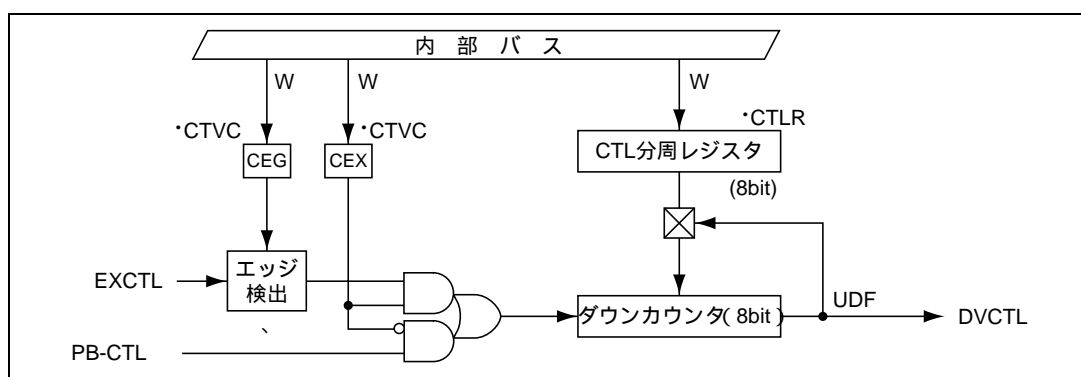
図 26.63 CTL 分周回路
