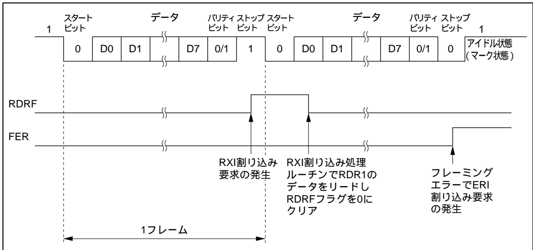
図 22.9 SCI の受信時の動作例 (8ビットデータ/パリティあり/1ストップビットの例)
