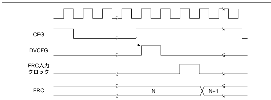
図 16.4 CFG クロック動作時のカウントタイミング
