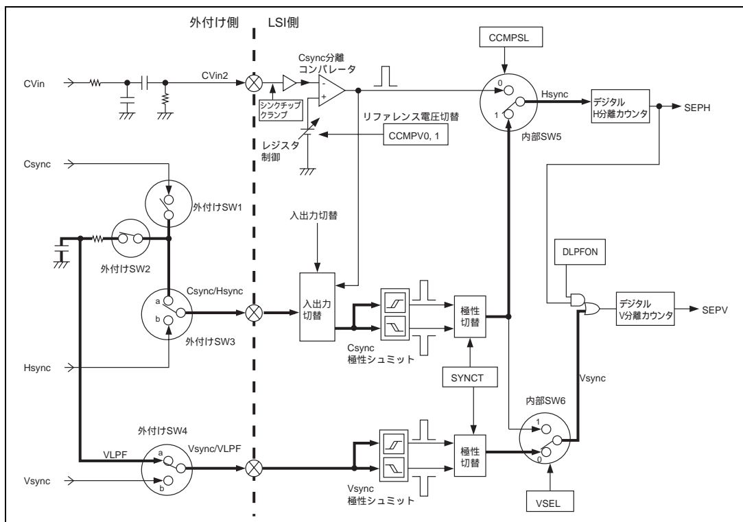
図 27.19 Csync 入力で Vsync シュミットを使用した場合の分離入力
