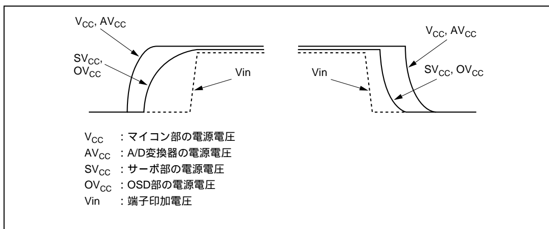
図 E.1 電源の立ち上げ・立ち下げの順序
