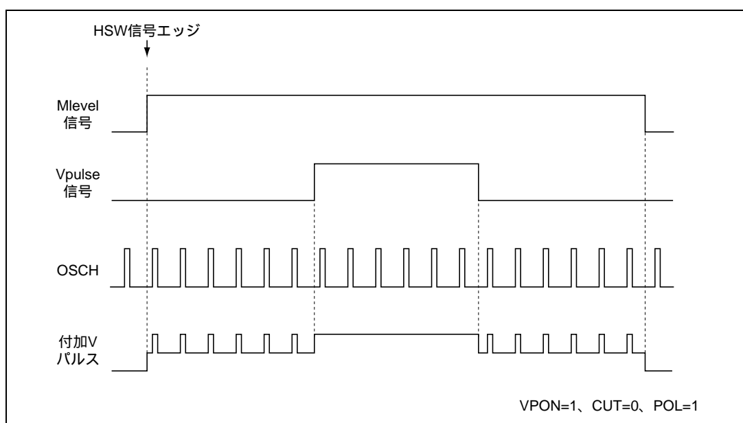
図 26.45 正極を指定したときの付加Vパルス
