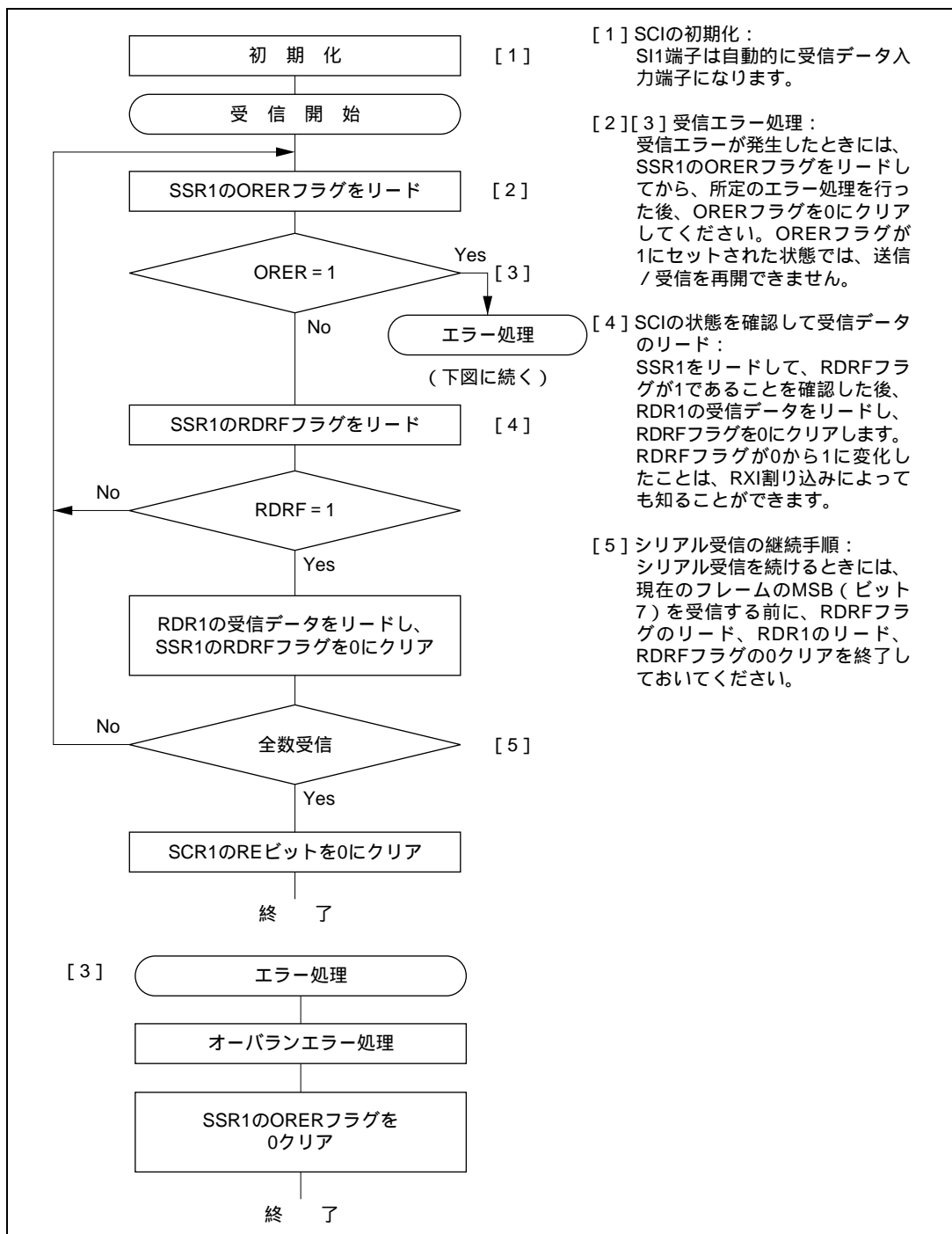
図 22.20 シリアルデータ受信フローチャートの例
