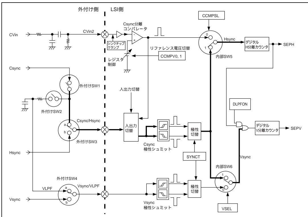
図 27.20 Csync 入力 で Csync シュミットを使用した場合の分離入力
