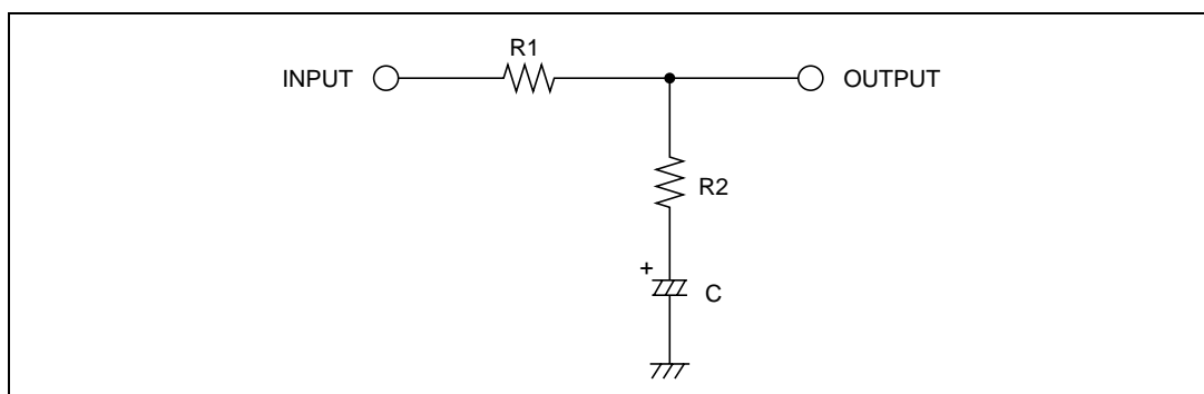
図 26.40 ラグリードフィルタ
