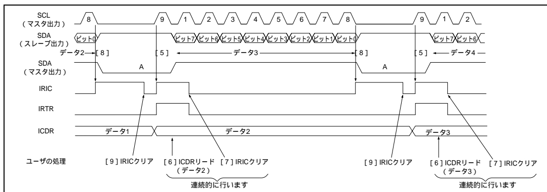
図 23.8 マスタ受信モード動作タイミング例 (MLS=ACKB=0、WAIT=1 のとき) (続き)
