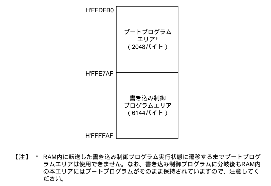
図 7.10 ブートモード時の RAM エリア
