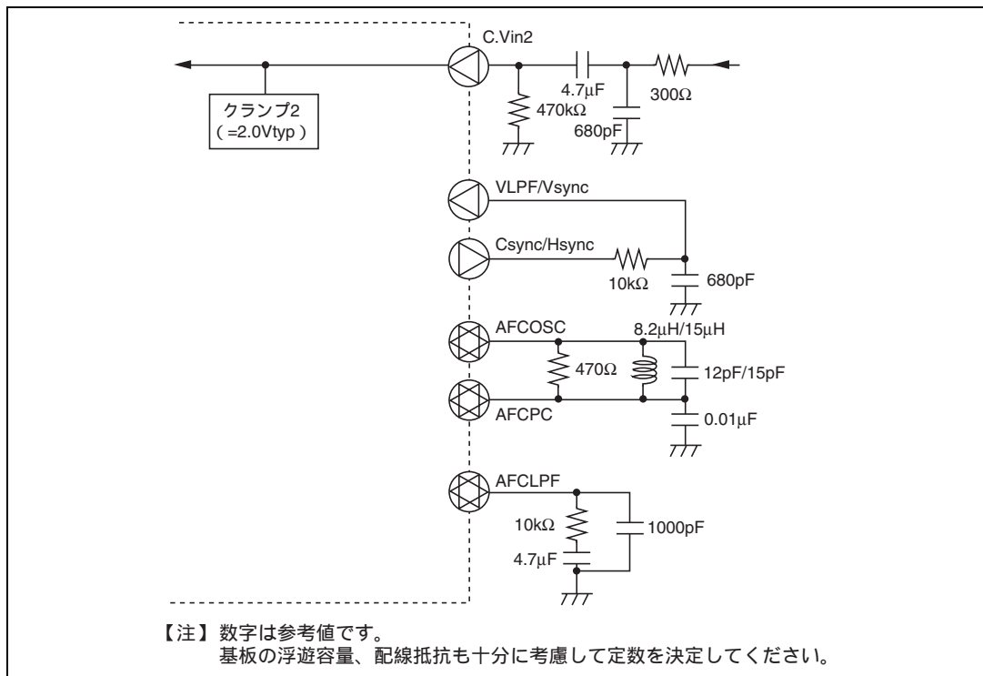
図 E.8 同期分離・データスライサ部の外部回路例 ( (1)CVin2 からの同期分離 )
