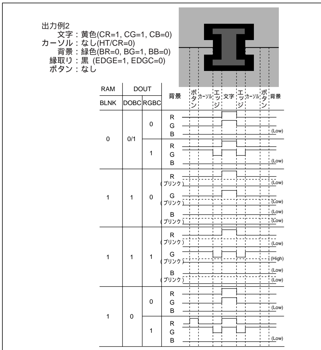
図 29.13 RGB 出力例 ( 2 )
