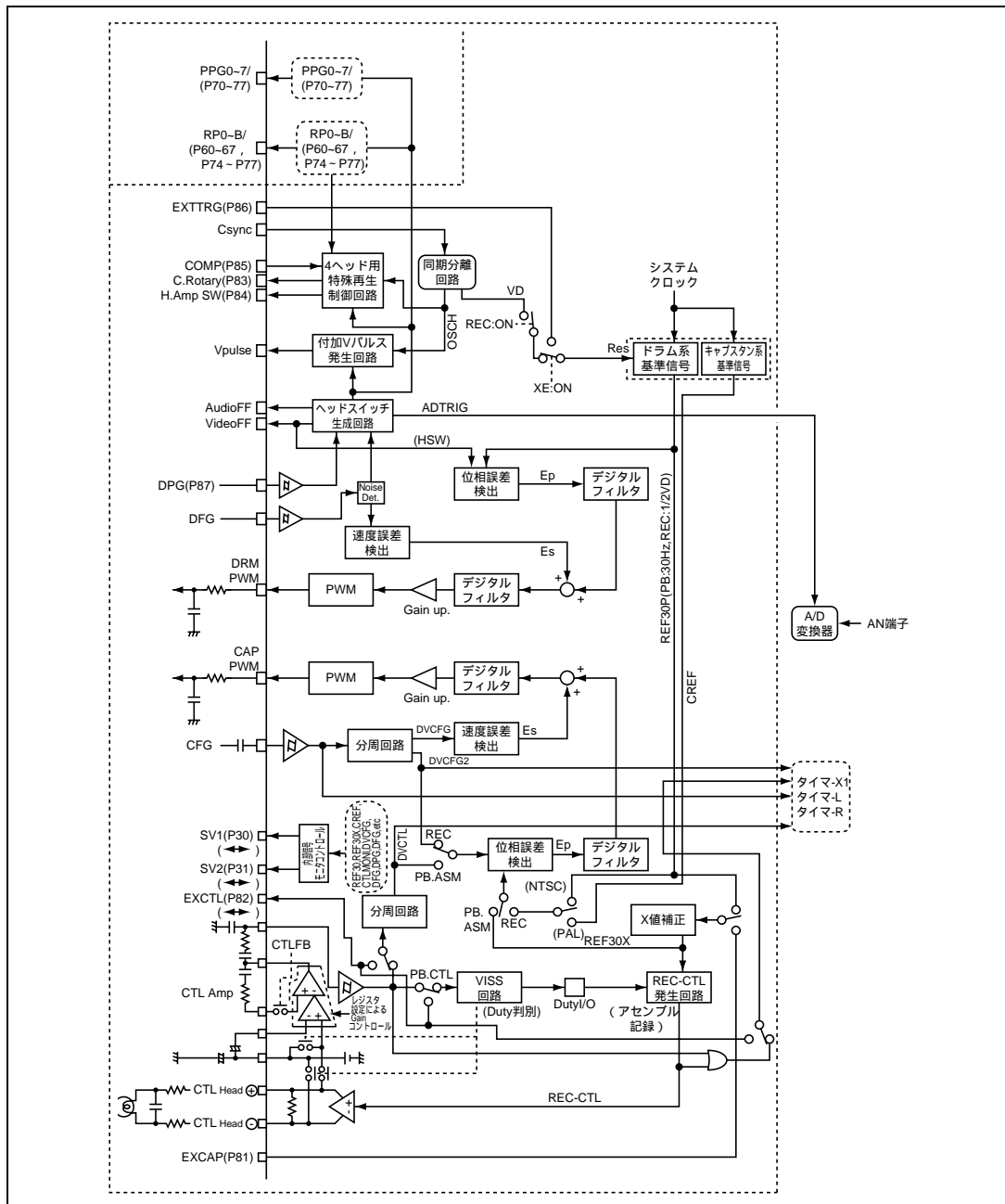
図 26.1 サーボブロック図
