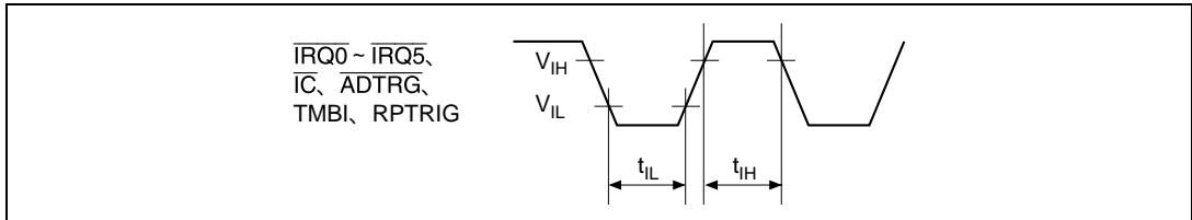
図 31.12 入力タイミング
