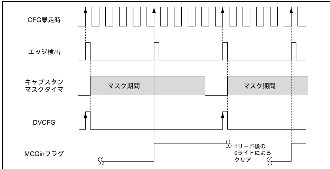
図 26.68 CFG マスクタイマの動作例 (キャプスタンモータ暴走時)
