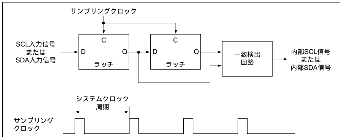
図 23.13 ノイズ除去回路のブロック図
