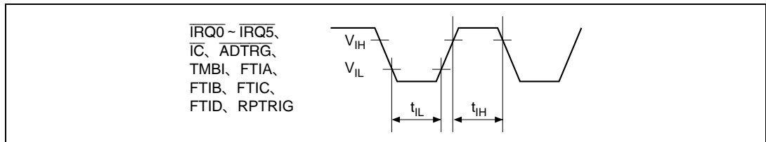
図 31.20 入力タイミング
