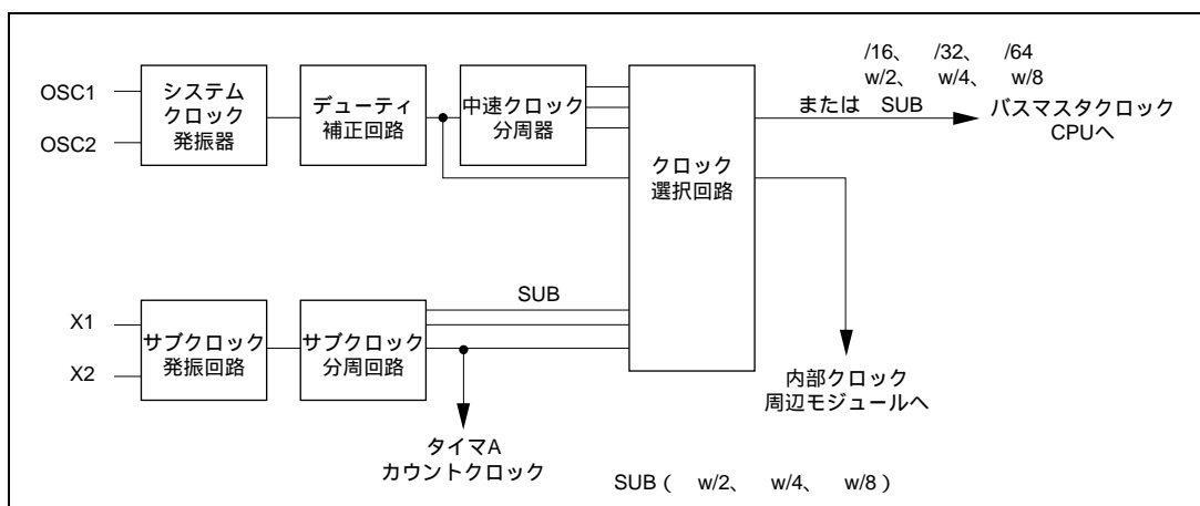
図 9.1 クロック発振器のブロック図
