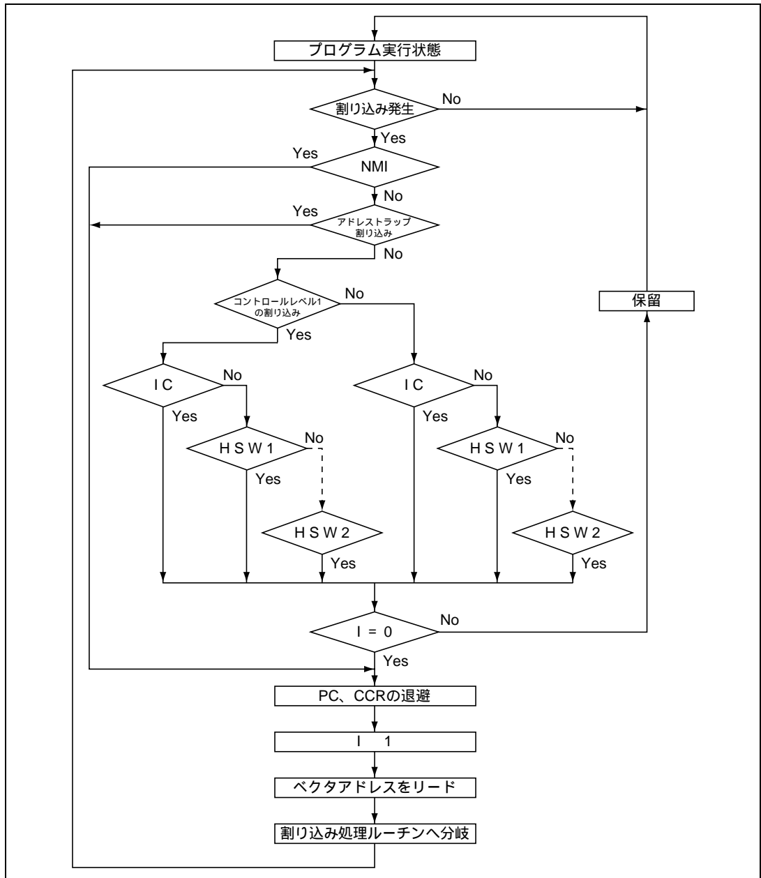
図 6.5 割り込み制御モード 0 の割り込み受けつけまでのフロー
