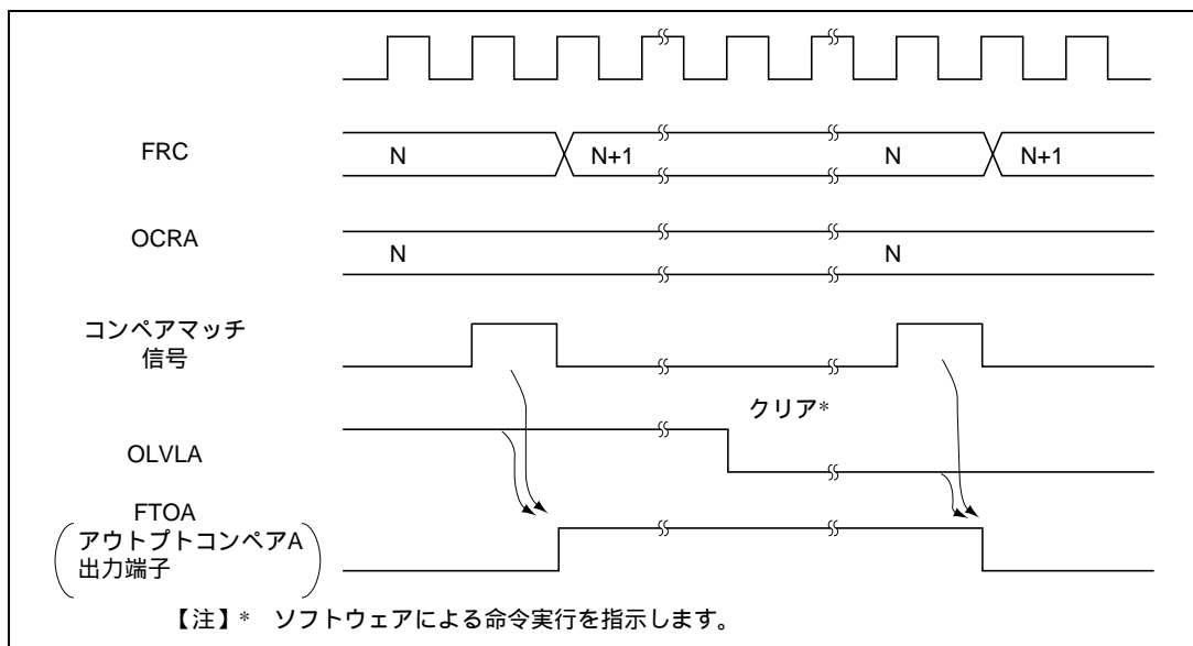
図 16.5 アウトプットコンペア A 出力タイミング
