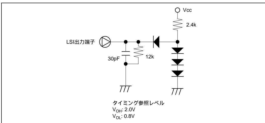
図 31.15 出力負荷条件
