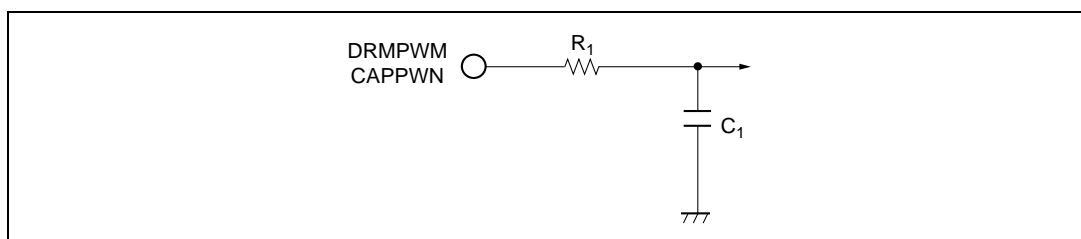
図 E.5 サーボ部の外付回路例
