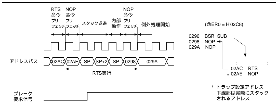
図 25.15 RTS 命令
