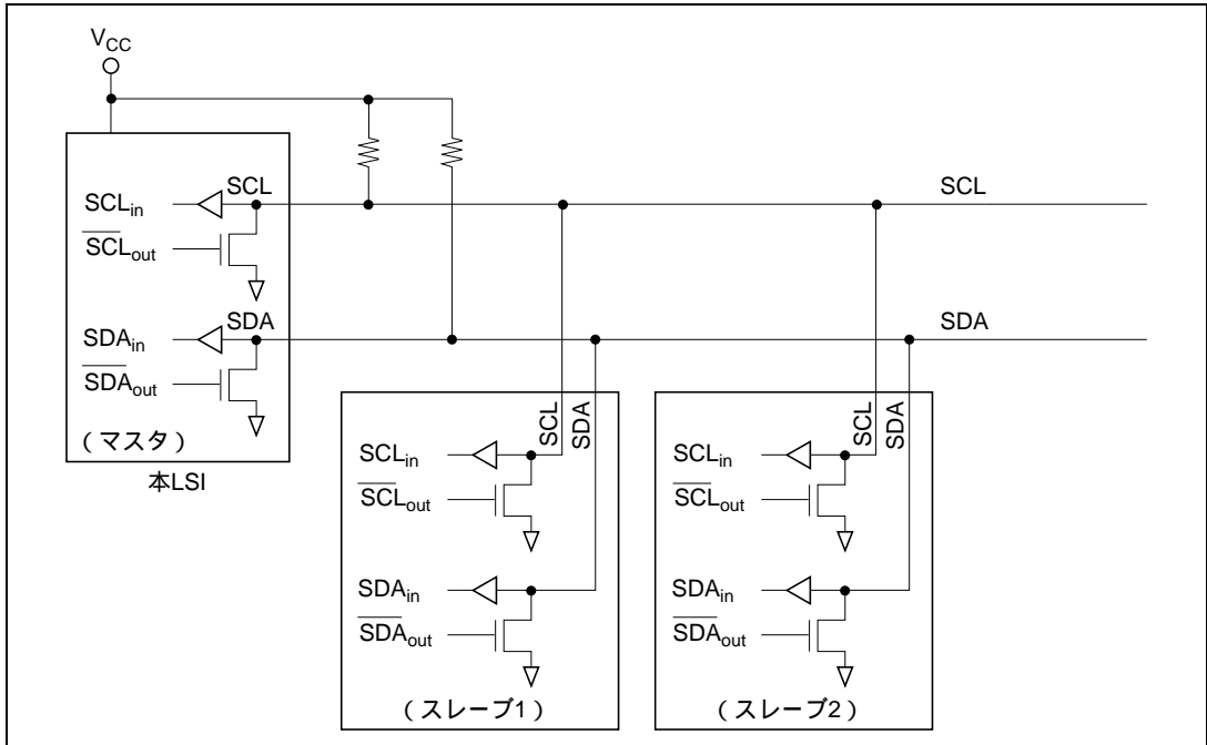
図 23.2 I 2 C バスインタフェース接続例 (本 LSI がマスタの場合)
