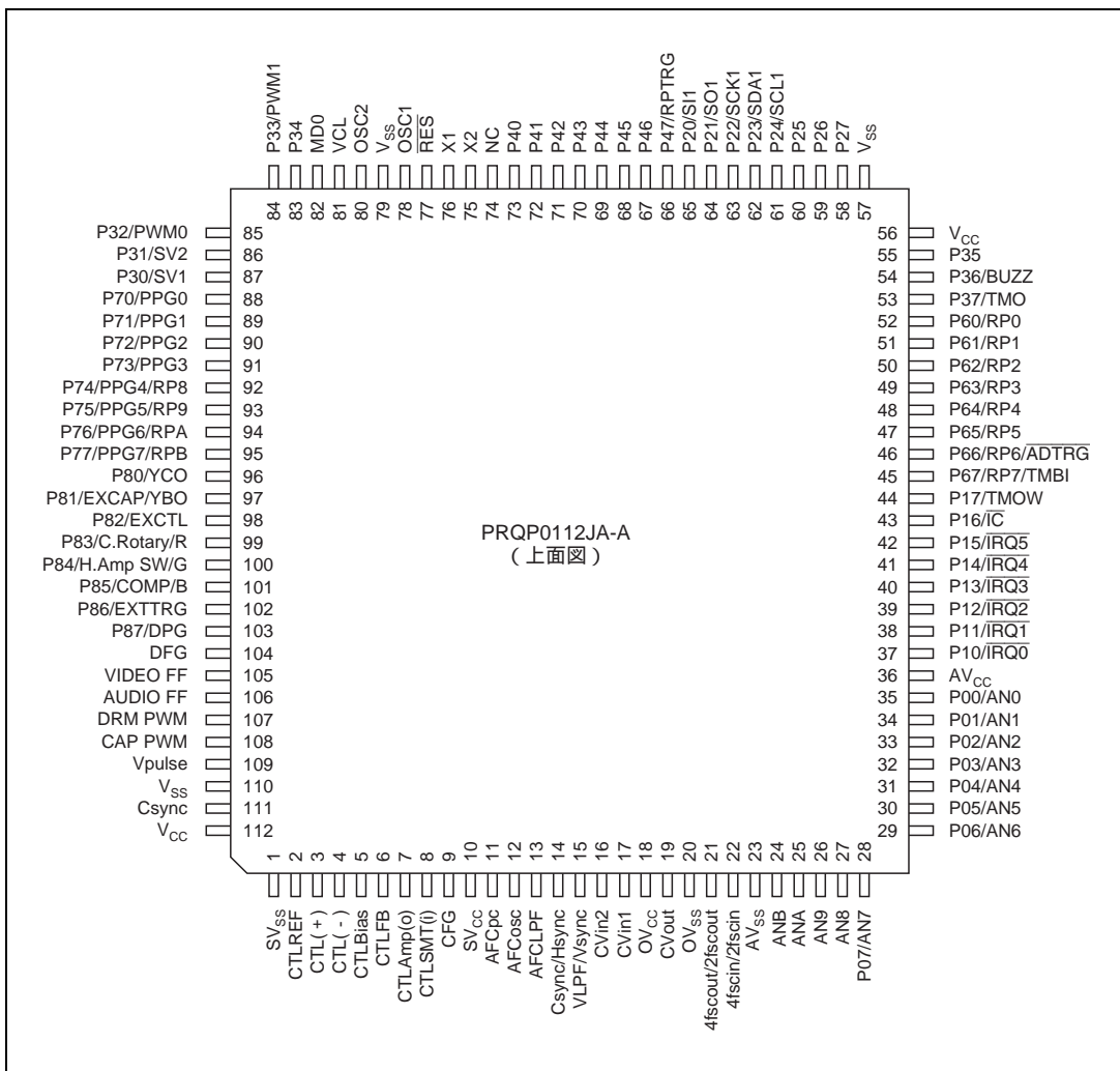
図 1.4 ピン配置図 (H8S/2197S、H8S/2196S)
