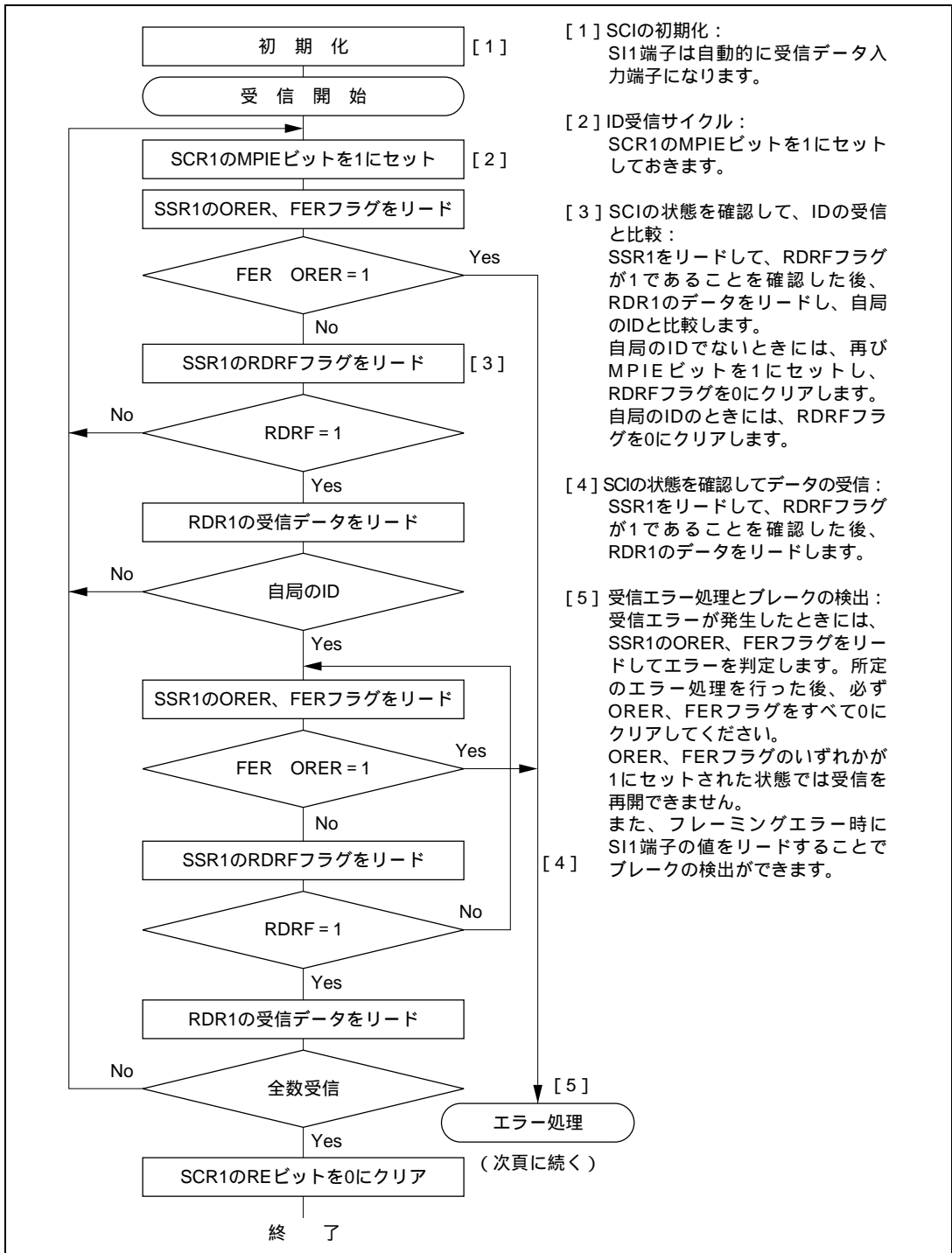
図 22.13 マルチプロセッサシリアル受信のフローチャートの例 (1)
