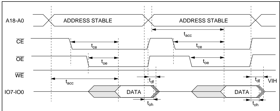
図 7.19 \overline{CE} 、 \overline{OE} クロック方式リード時のタイミング波形
