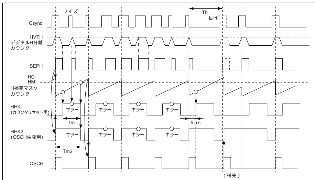
図 27.14 H 補完マスクカウンタの補完とマスクタイミング
