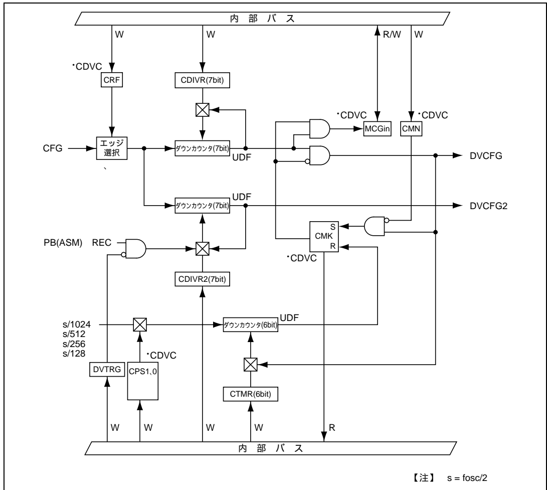
図 26.65 CFG 分周回路
