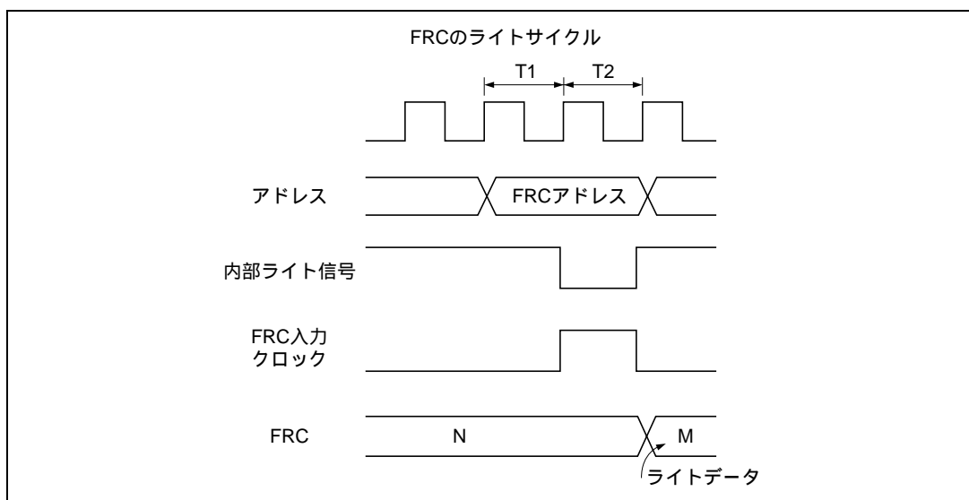
図 16.14 FRC のライトとカウントアップの競合
