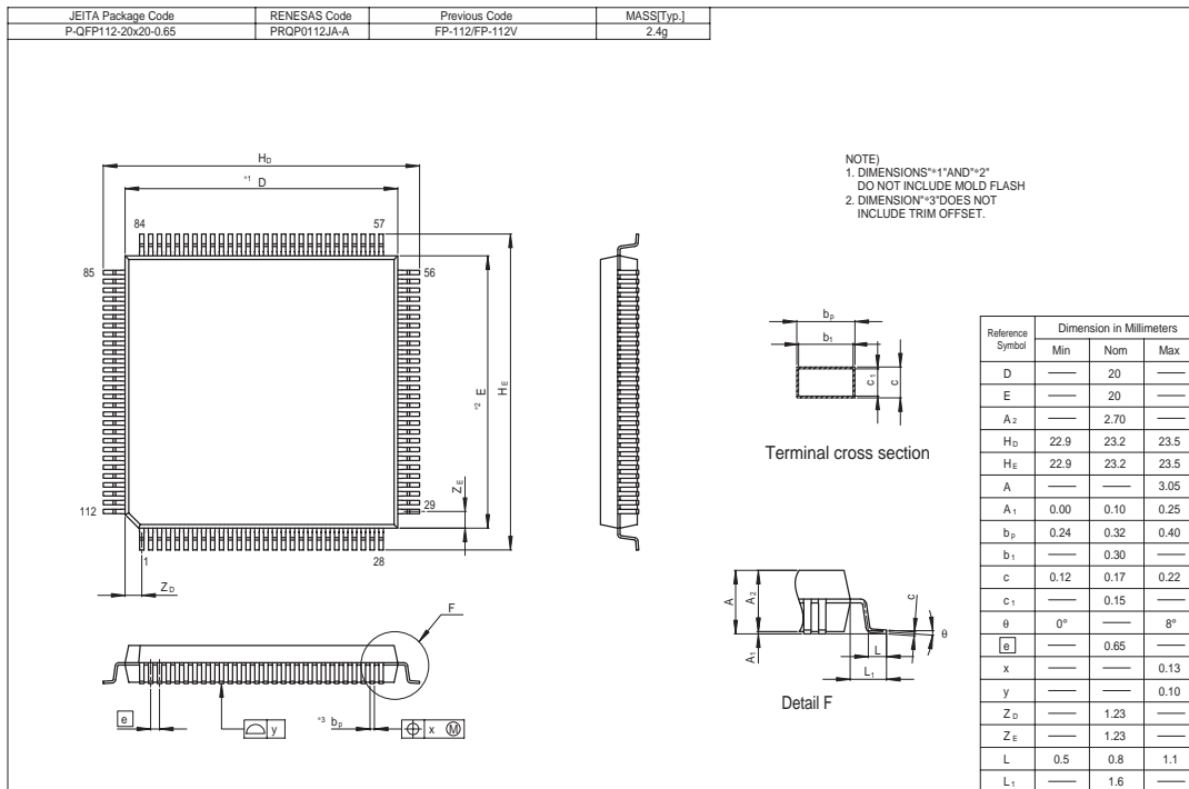
図 H.1 外形寸法図 (PRQP0112JA-A)
