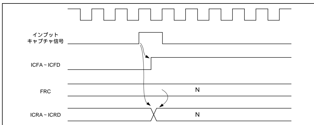
図 16.9 ICFA ~ ICFD のセットタイミング
