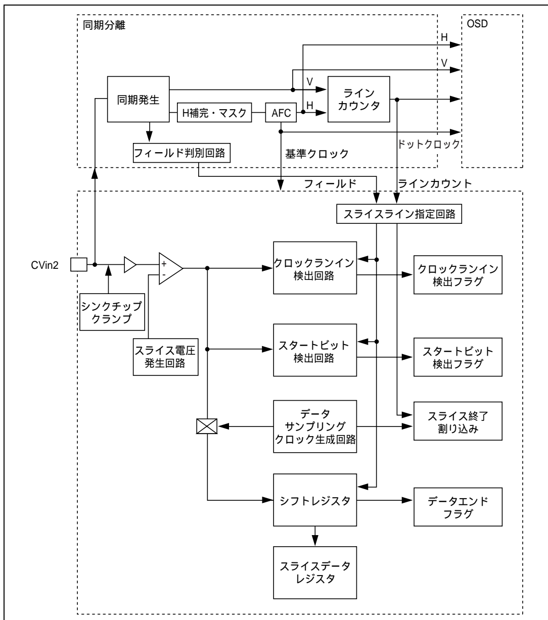
図 28.1 データスライサブロック図
