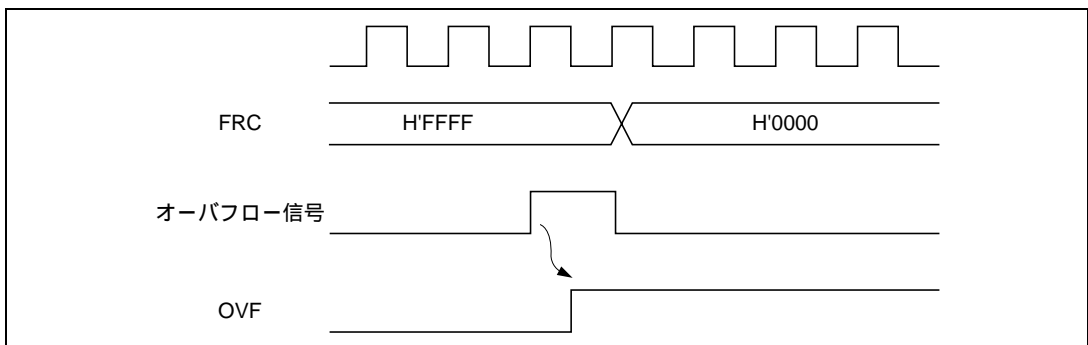
図 16.11 OVF セットタイミング
