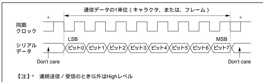
図 22.16 クロック同期式通信のデータフォーマット
