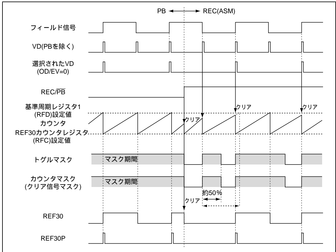
図 26.17 PB REC 切り替え時の基準信号の生成 (2)
