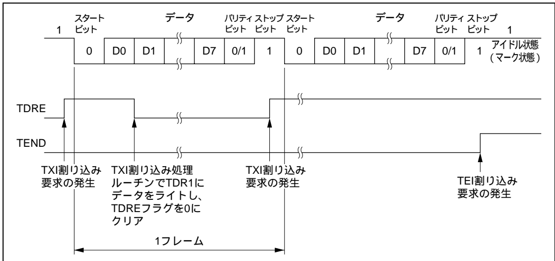
図 22.6 調歩同期式モードでの送信時の動作例 (8ビットデータ/パリティあり/1ストップビットの例)
