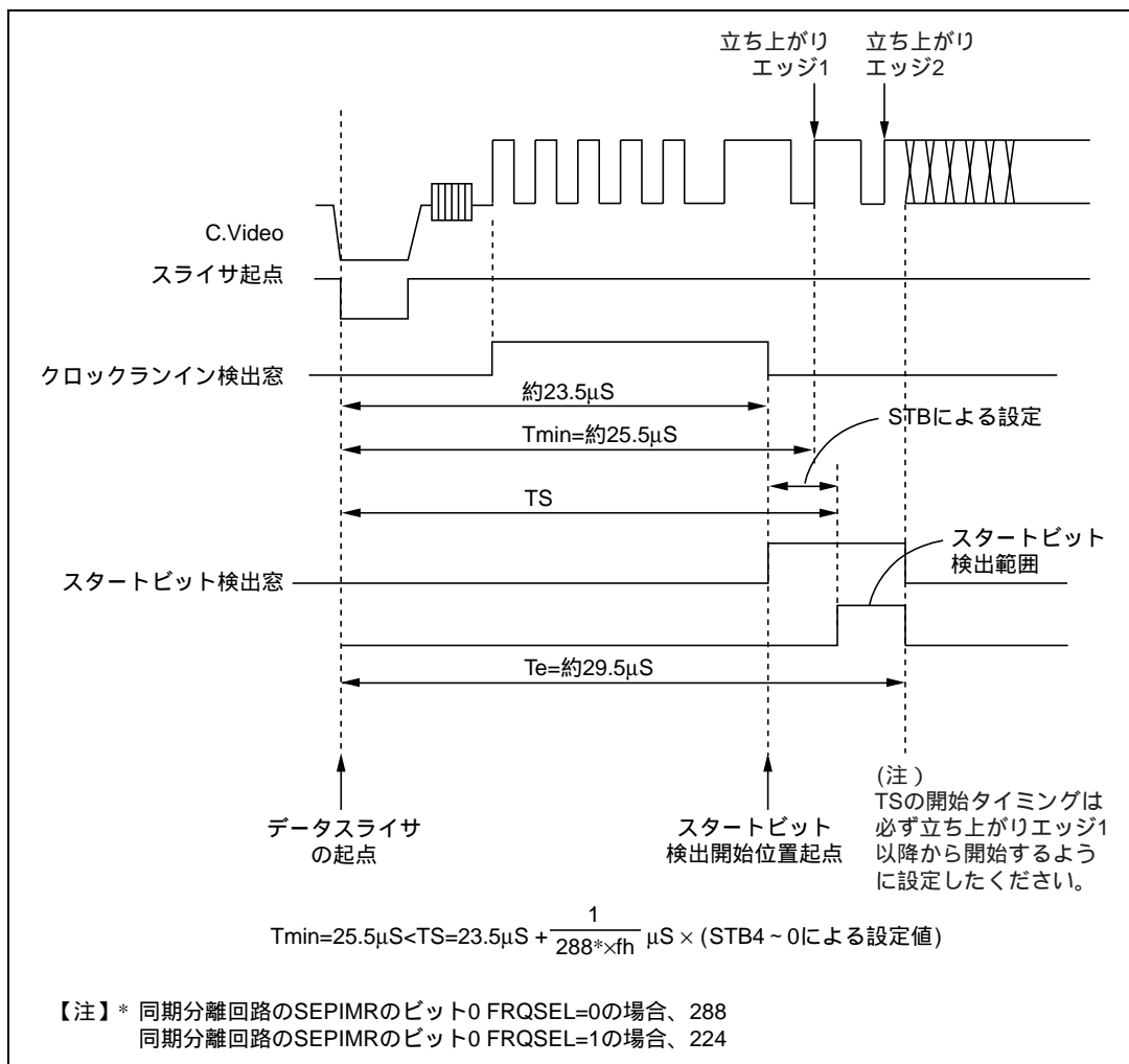
図 28.12 DSL32B ビットを 1 にセットした場合のスタートビット検出開始位置
