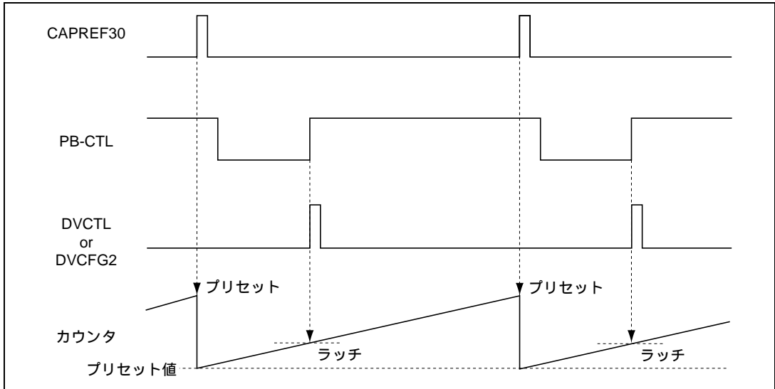
図 26.35 再生時のキャプスタン位相制御
