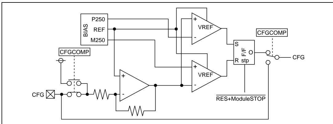
図 26.3 CFG 入力回路
