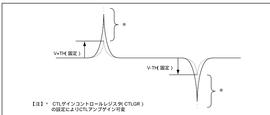
図 26.53 CTL 入力パルスのゲインコントロール概念
