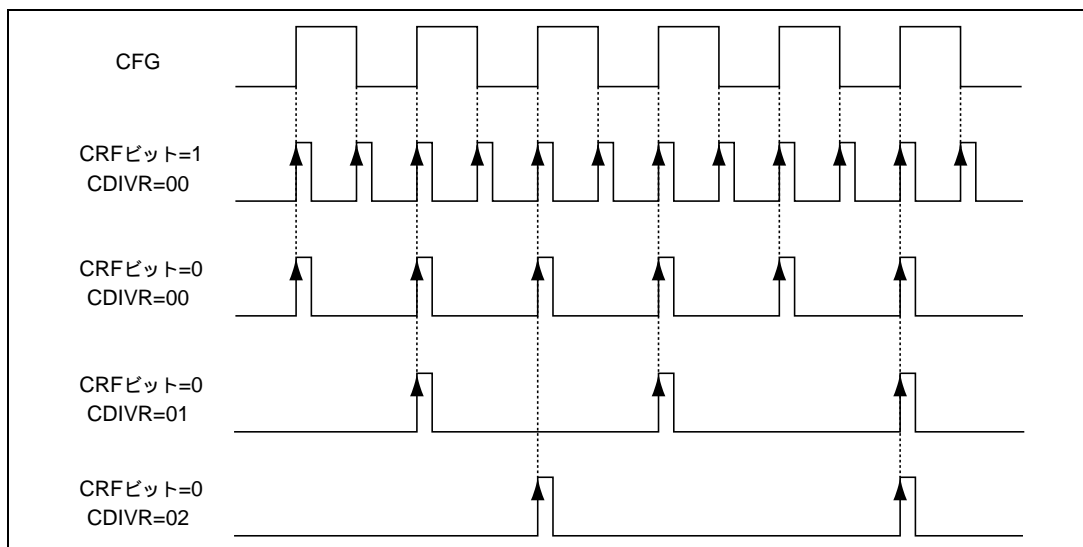
図 26.66 CFG 分周波形例
