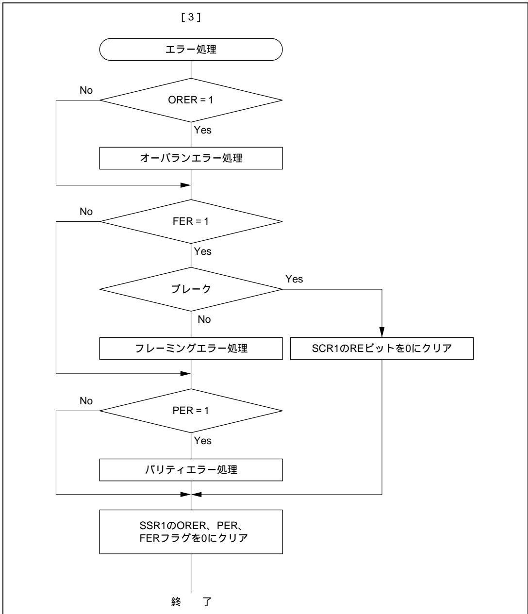
図 22.8 シリアル受信データフローチャートの例 (2)
