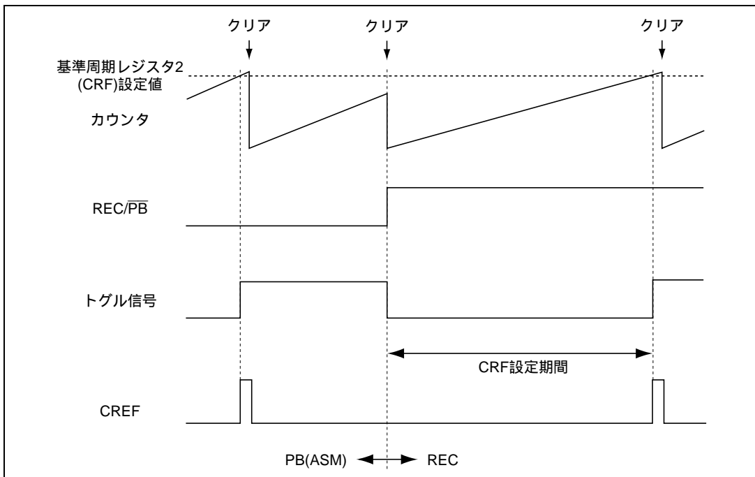
図 26.14 PB REC時のCREF信号 (CRDビット=0の時)
