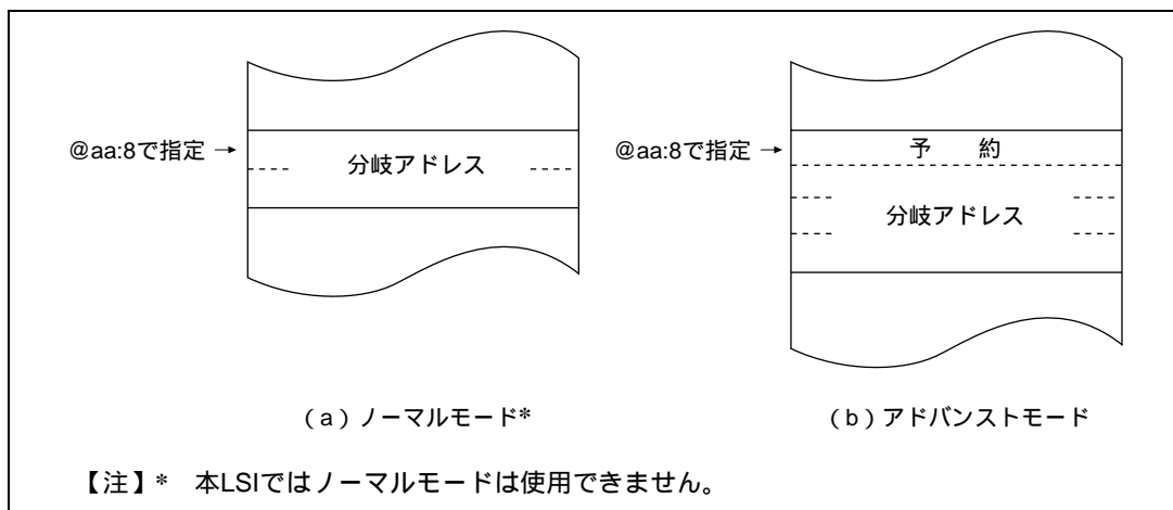
図 2.14 メモリ間接による分岐アドレスの指定
