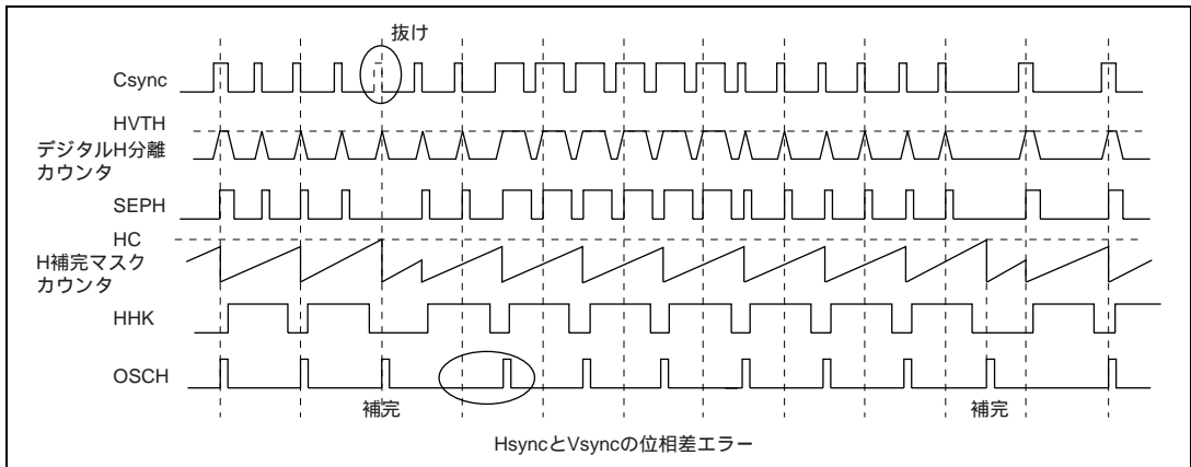
図 27.5 Hsync 位置にある等価パルス抜け発生時の Hsync と Vsync の位相差エラー発生タイミング
