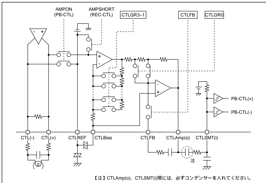
図 26.4 CTL 入力回路
