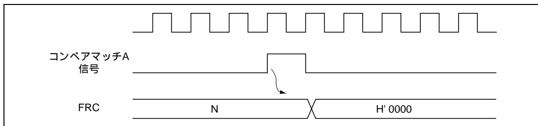
図 16.6 コンペアマッチ A によるクリアタイミング
