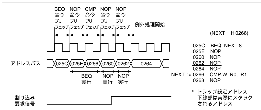
図 25.9 Bcc 命令で条件不成立時 (分岐先にトラップアドレス)
