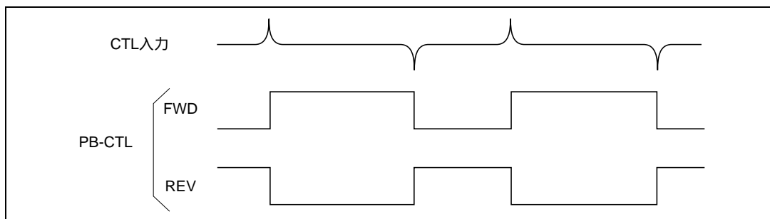
図 26.48 FWD/REV 時の PB-CTL 信号
