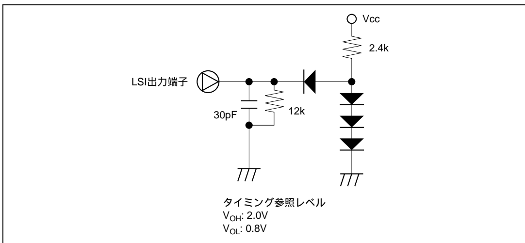
図 31.7 出力負荷条件
