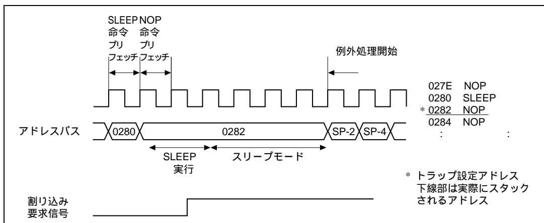
図 25.18 SLEEP 命令 (3)
