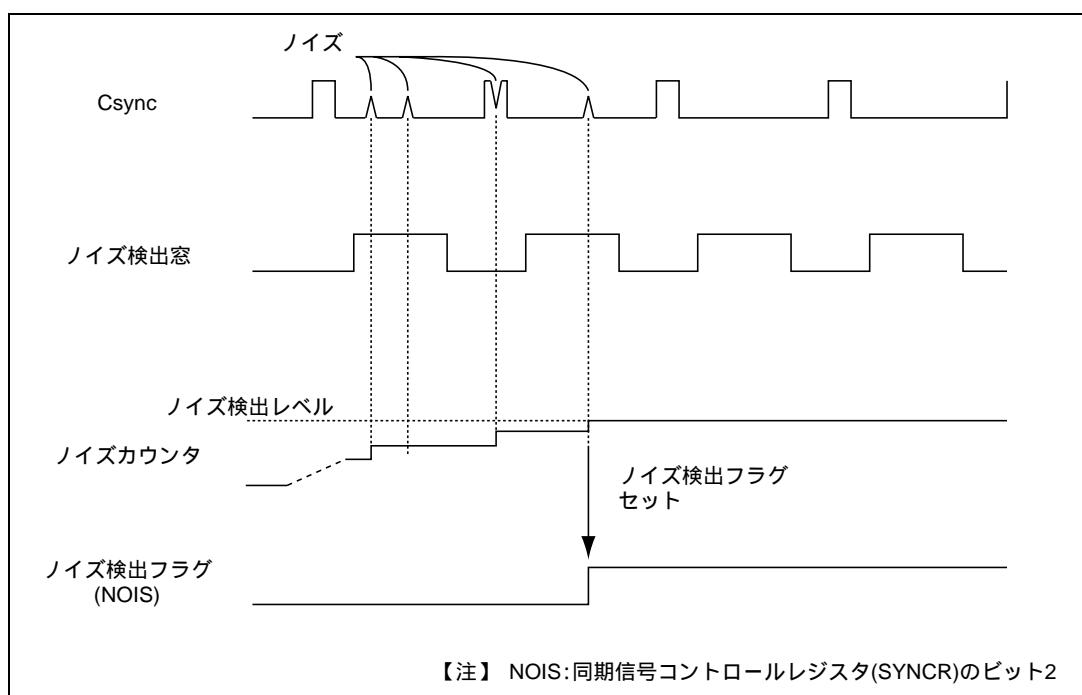
図 26.76 ノイズ検出動作
