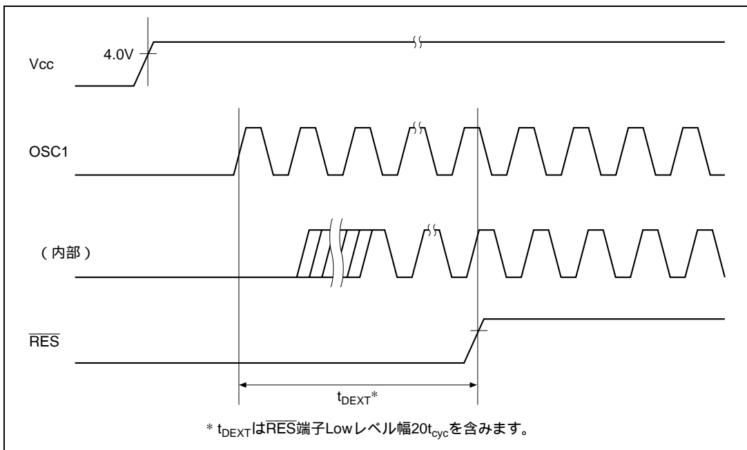
図 31.18 外部クロック安定遅延時間タイミング
