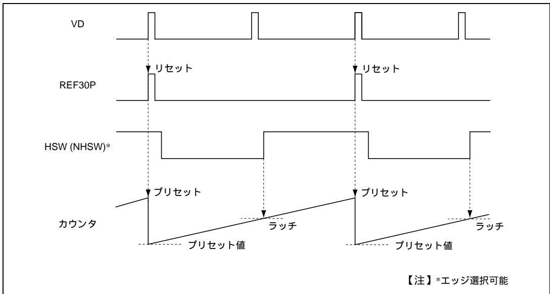
図 26.31 記録時のドラム位相制御 (HSW 立ち上がりエッジを選択)
