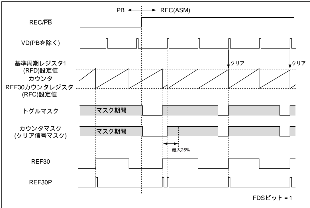
図 26.20 RFD ビット=1 の時、PB REC 切り替え時の基準信号の生成 (3)
