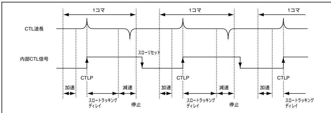
図 26.54 スローモード時の PB-CTL 波形
