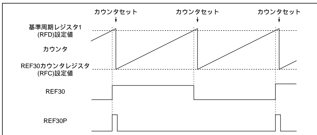
図 26.8 再生時の REF30 信号
