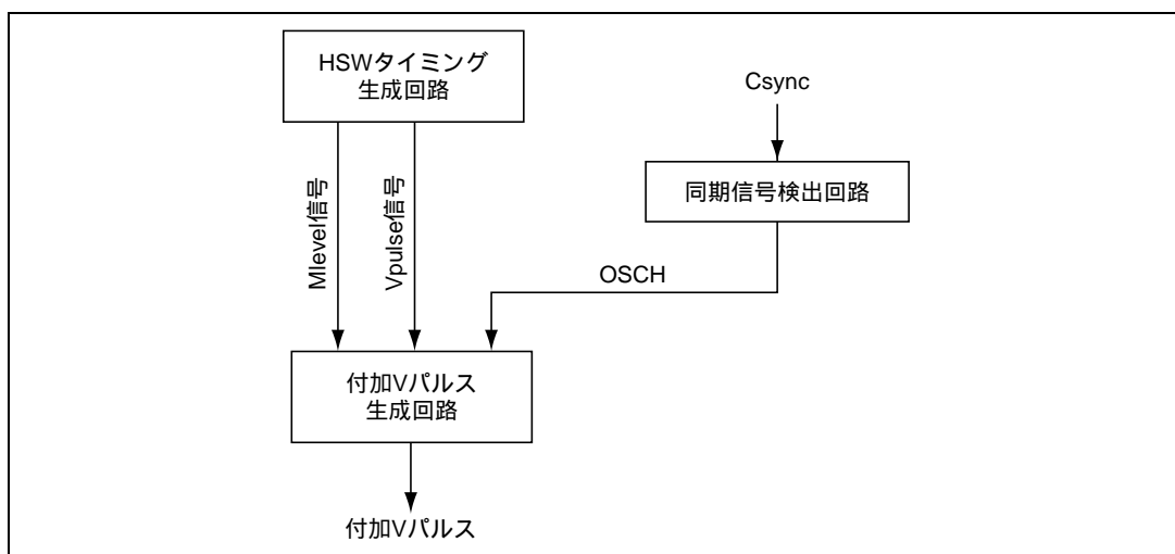
図 26.43 付加 V パルス制御回路
