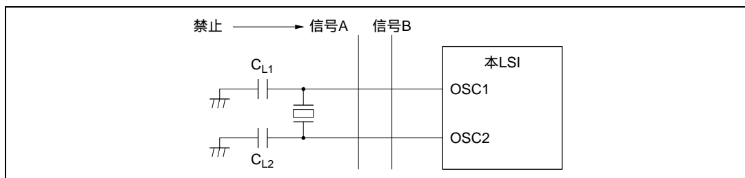
図 9.4 発振回路部のボード設計に関する注意事項
