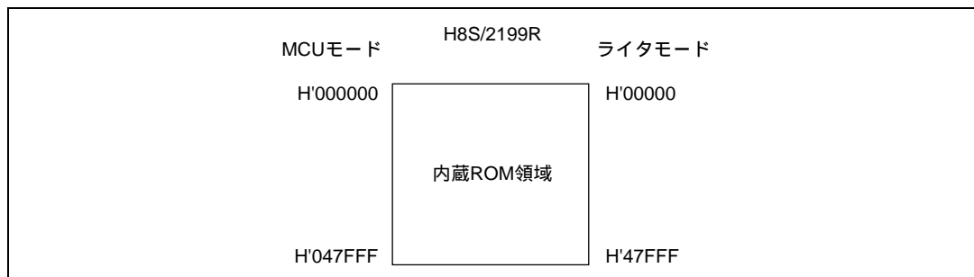
図 7.15 ライターモード時のメモリマップ
