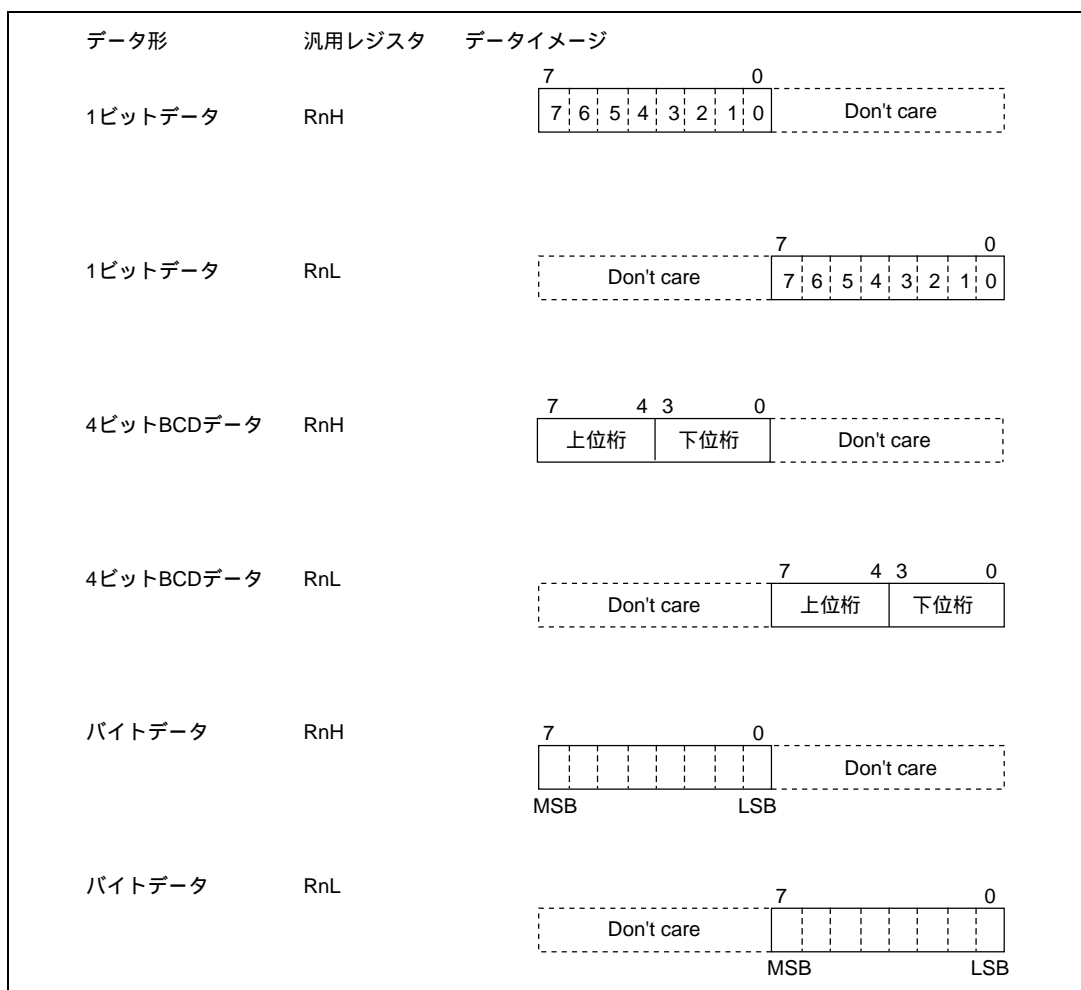
図2.10 汎用レジスタのデータ構成（1）
