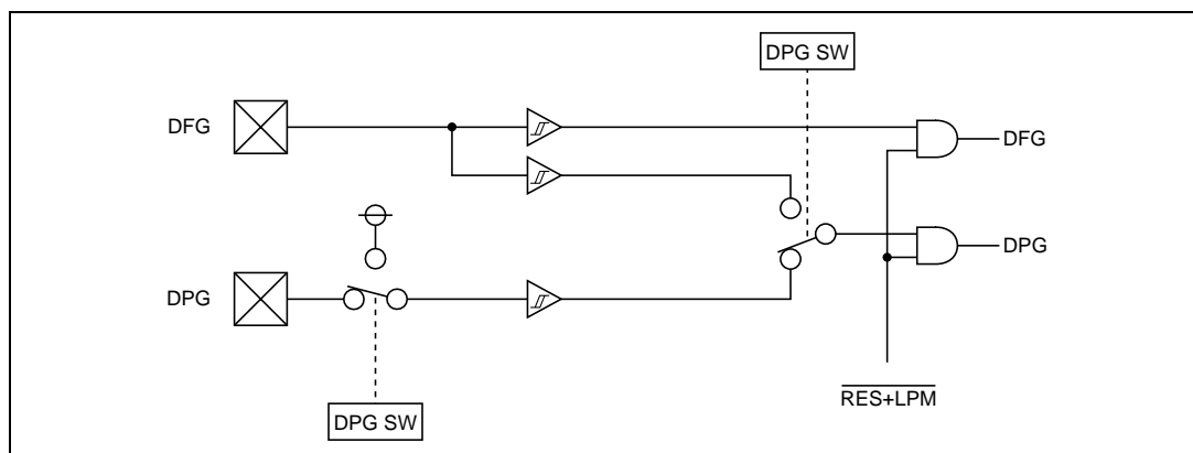
図 26.2 DFG、DPG 入力回路
