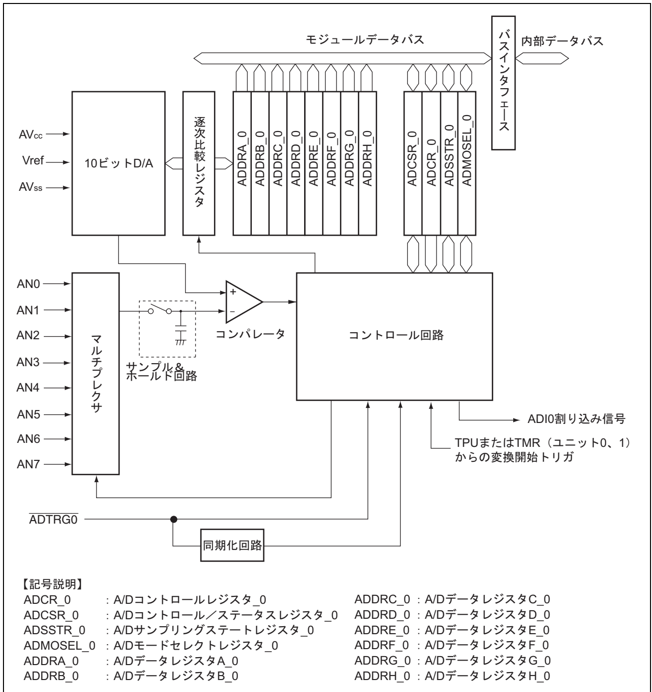
図 19.1 A/D 変換器 (ユニット 0/AD_0) のブロック図
