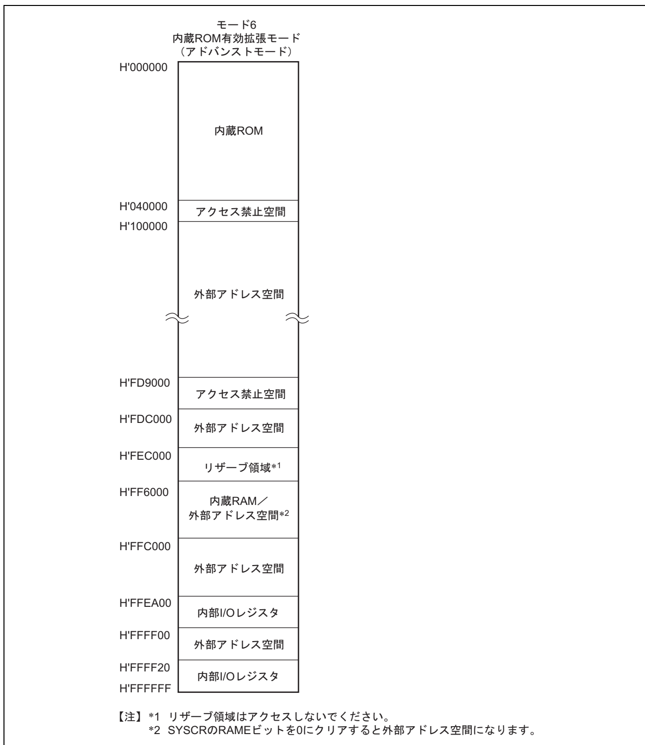
図 3.3 H8SX/1631、H8SX/1631L の各動作モードのアドレスマップ (2)
