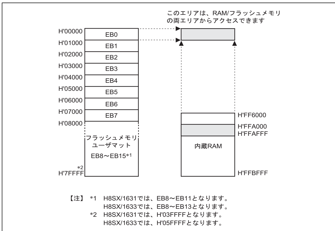
図 22.18 RAM のオーバーラップ動作例 (H8SX/1635)
