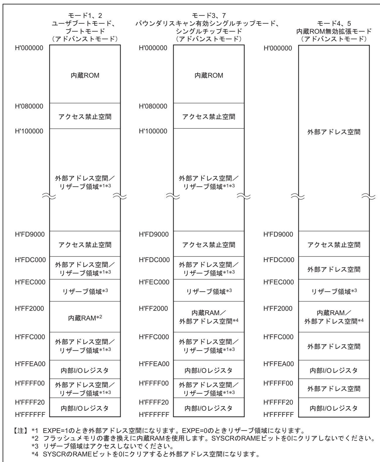
図 3.1 H8SX/1635、H8SX/1635L の各動作モードのアドレスマップ (1)
