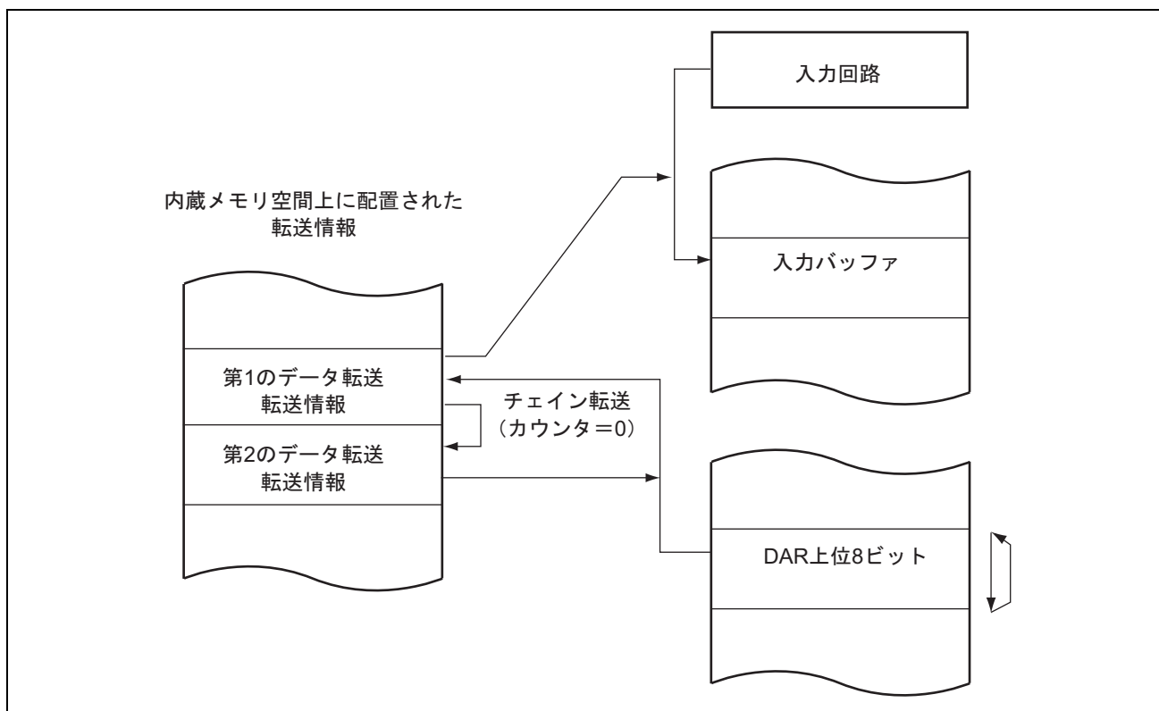
図 11.16 カウンタ=0 時のチェイン転送
