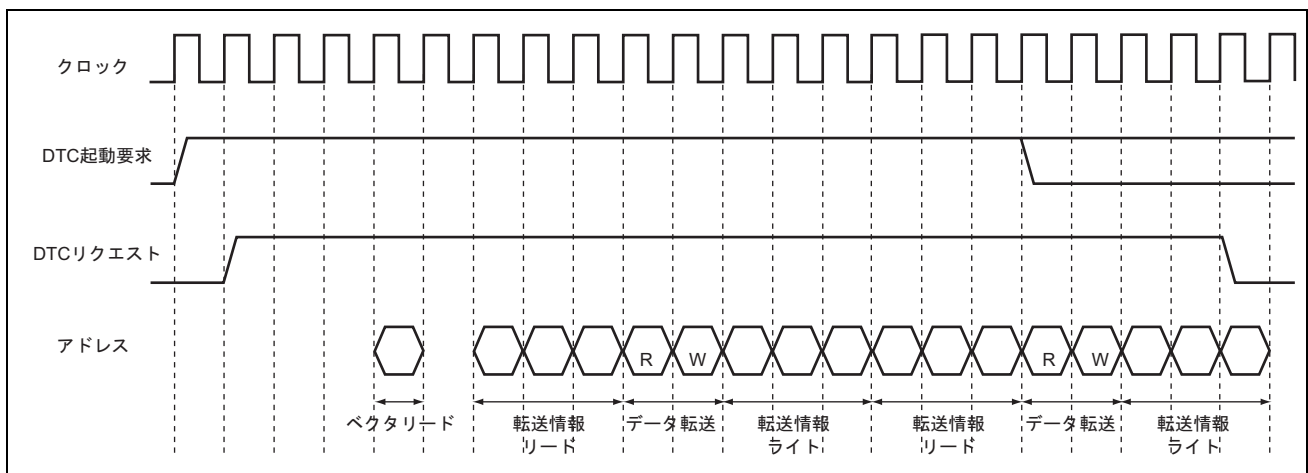
図 11.13 DTC の動作タイミング例 (ショートアドレスモード、チェーン転送)
