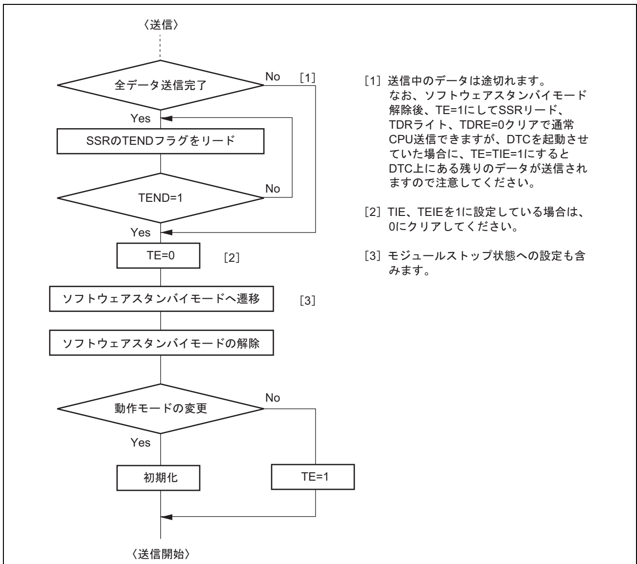
図 17.39 送信時のソフトウェアスタンバイモード遷移フローチャートの例
