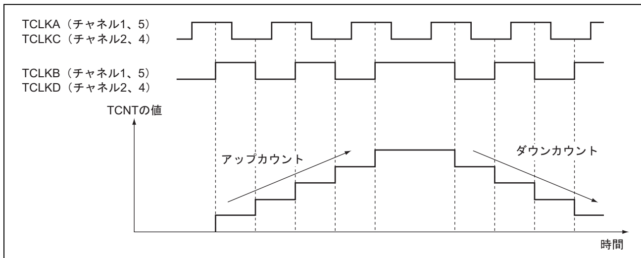
図 13.29 位相計数モード4の動作例
