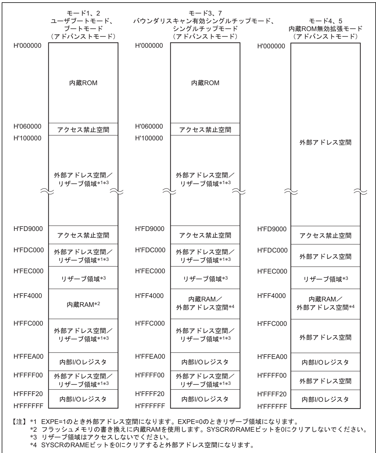
図 3.2 H8SX/1633、H8SX/1633L の各動作モードのアドレスマップ (1)
