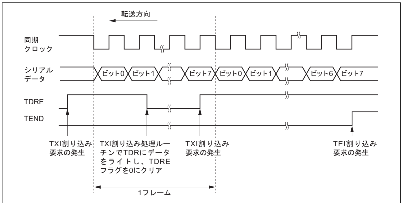
図 17.19 クロック同期式モードの送信時の動作例
