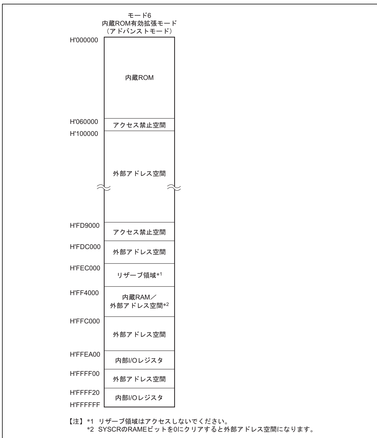
図 3.2 H8SX/1633、H8SX/1633L の各動作モードのアドレスマップ (2)
