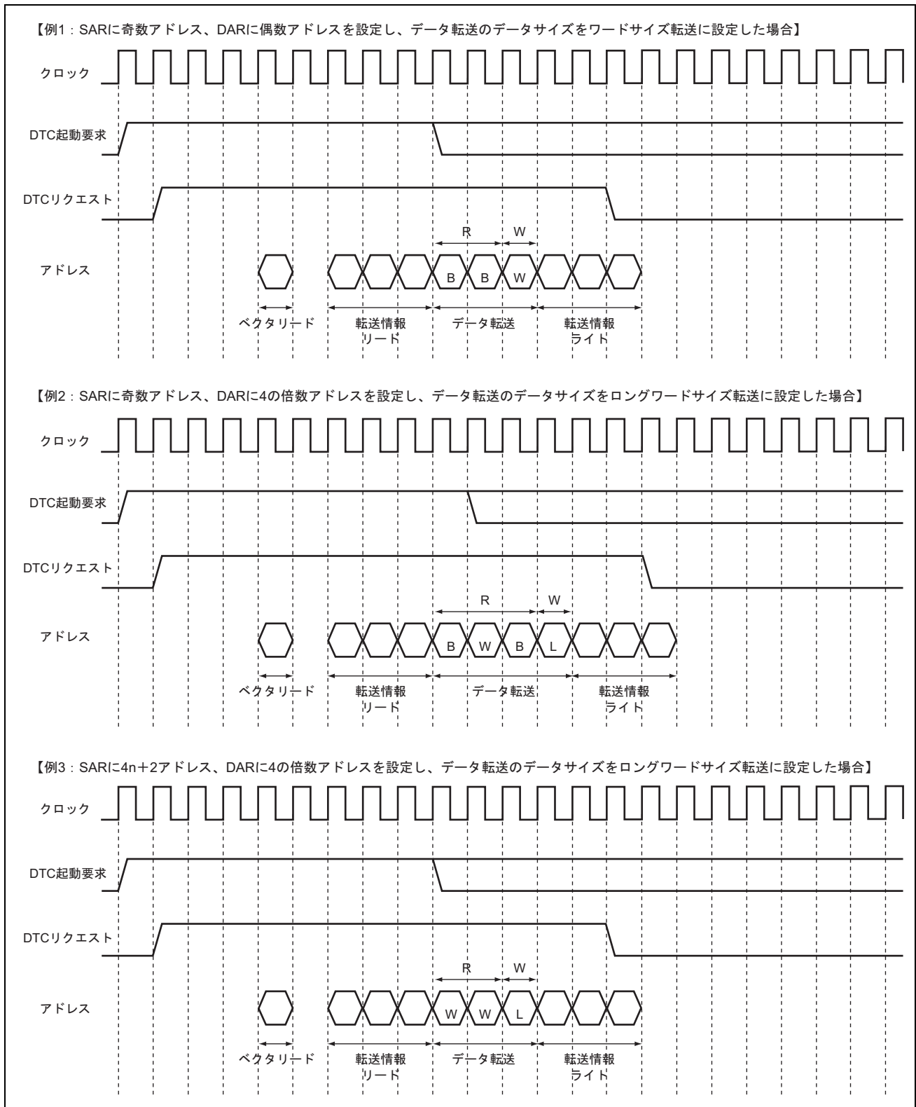
図 11.5 バスサイクルが分割される例
