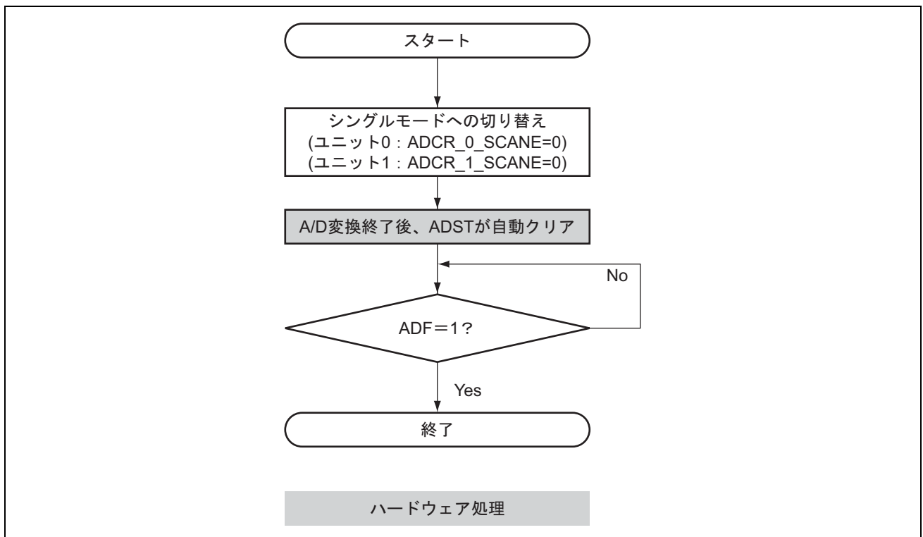
図 19.11 ソフトウェア起動による連続スキャンモード停止方法
