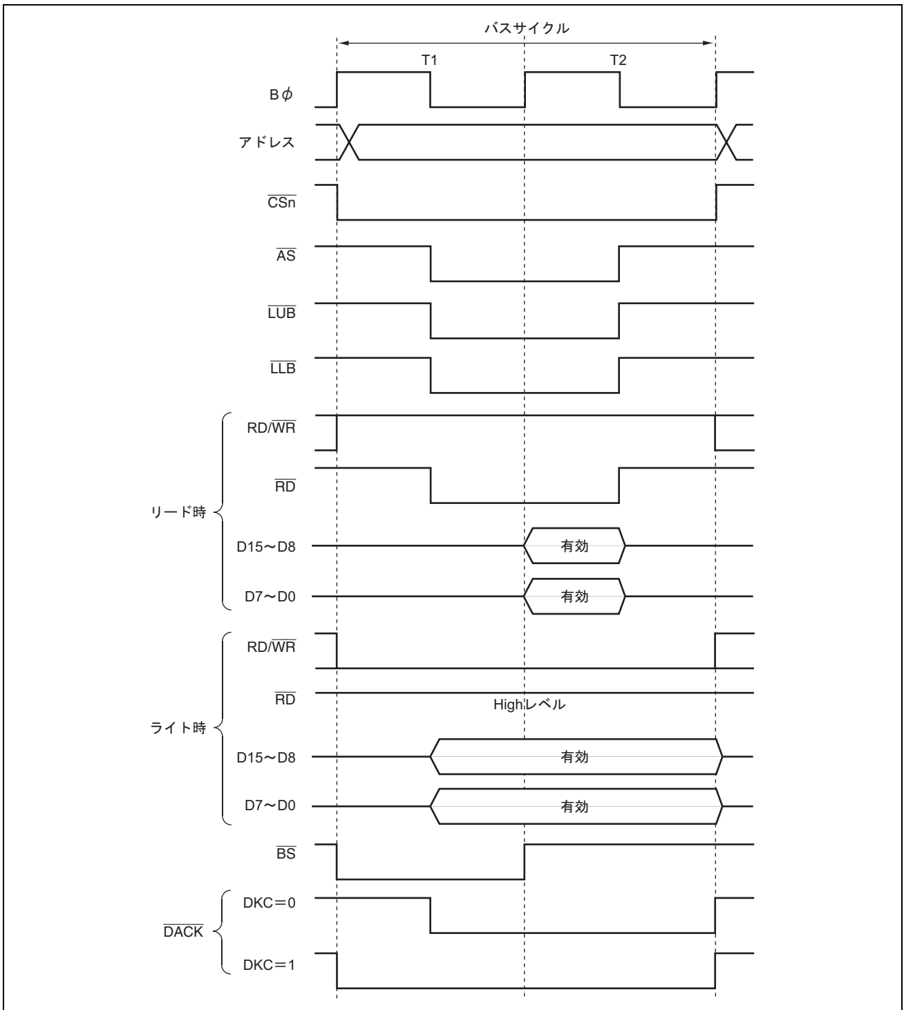
図 9.27 \overline{\text{DACK}} 信号の出カタイミング
