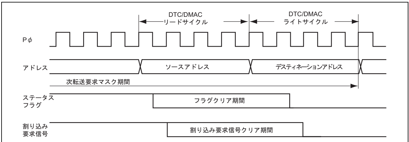
図 13.45 DTC/DMAC の起動によるステータスフラグのクリアタイミング例 (2)
