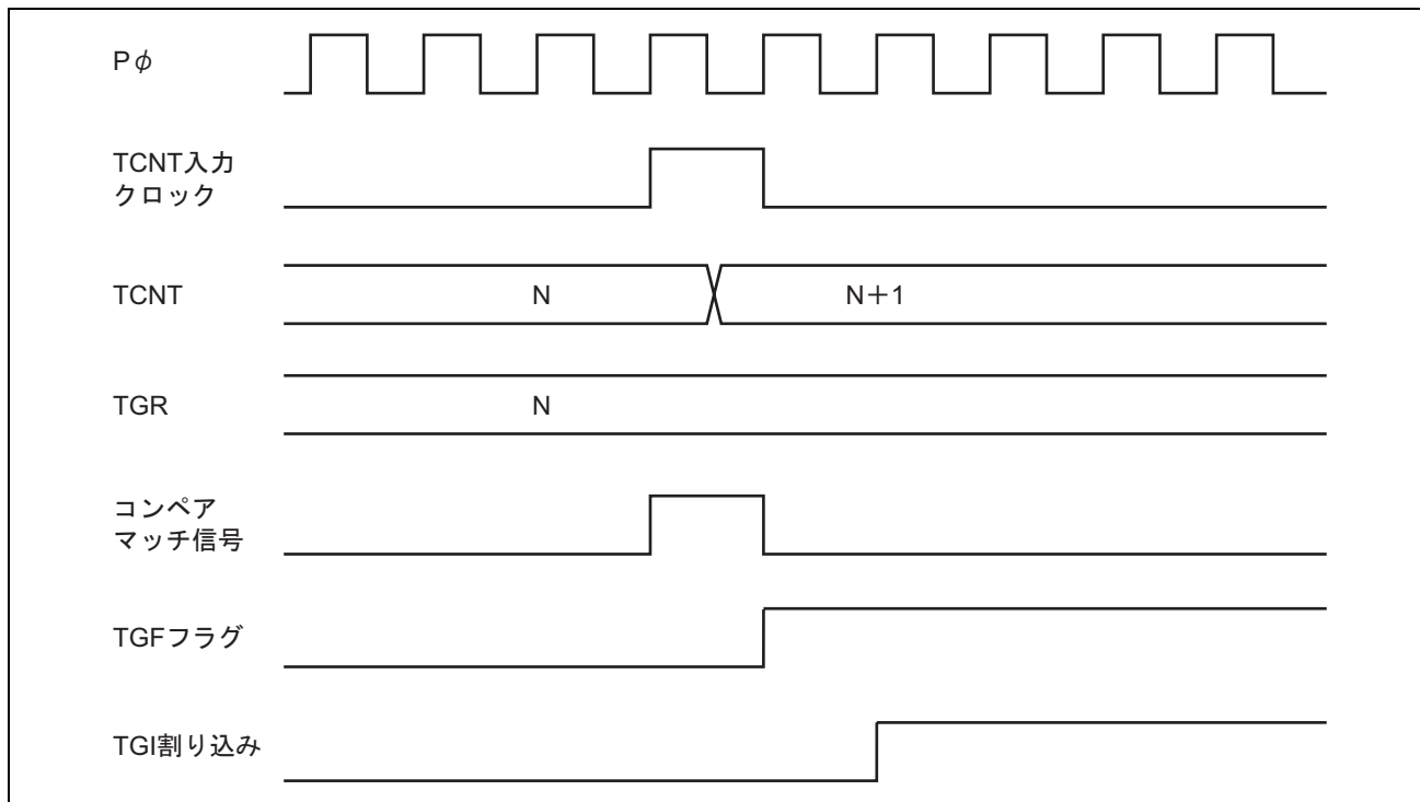
図 13.39 TGI 割り込みタイミング (コンペアマッチ)
