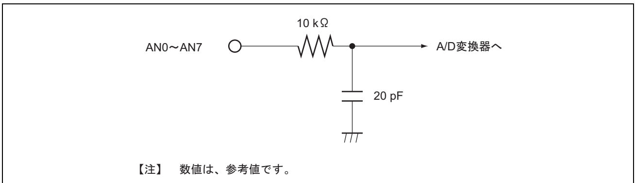
図 19.15 アナログ入力端子等価回路
