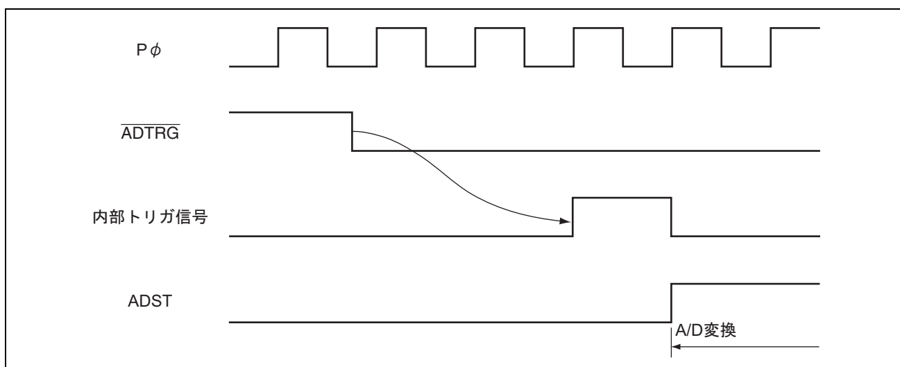
図 19.7 外部トリガ入力タイミング (TRGS1、TRGS0、EXTRGS≠B'111)
