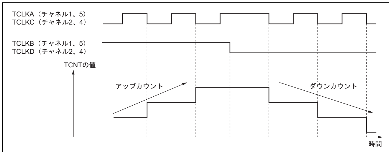
図 13.27 位相計数モード2の動作例
