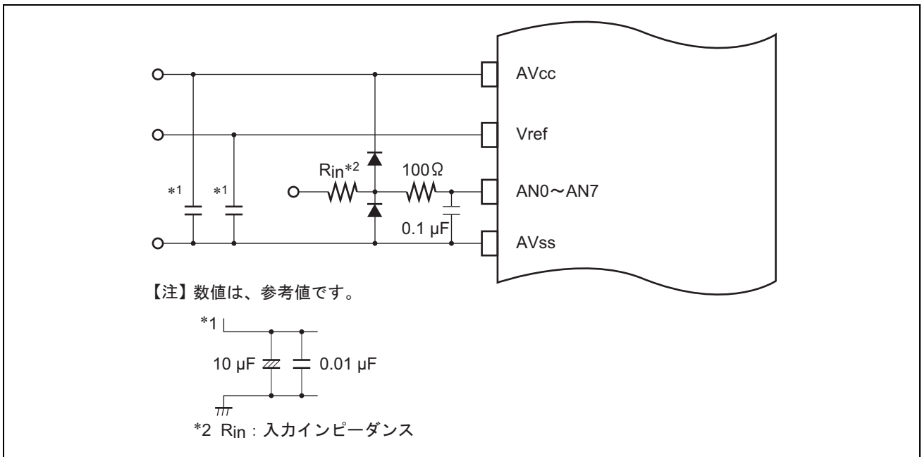
図 19.14 アナログ入力保護回路の例
