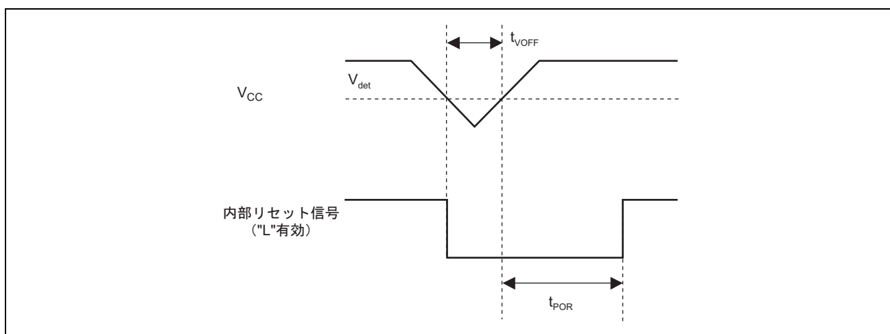
図 27.41 電圧検出回路タイミング
