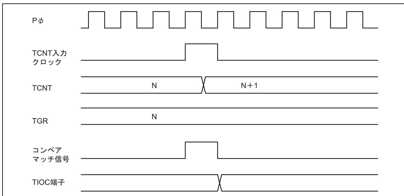
図 13.33 アウトプットコンペア出力タイミング
