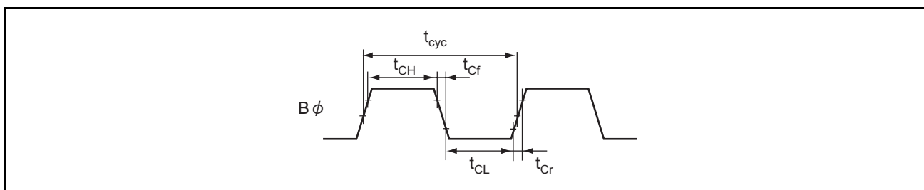
図 27.2 外部バスクロックタイミング
