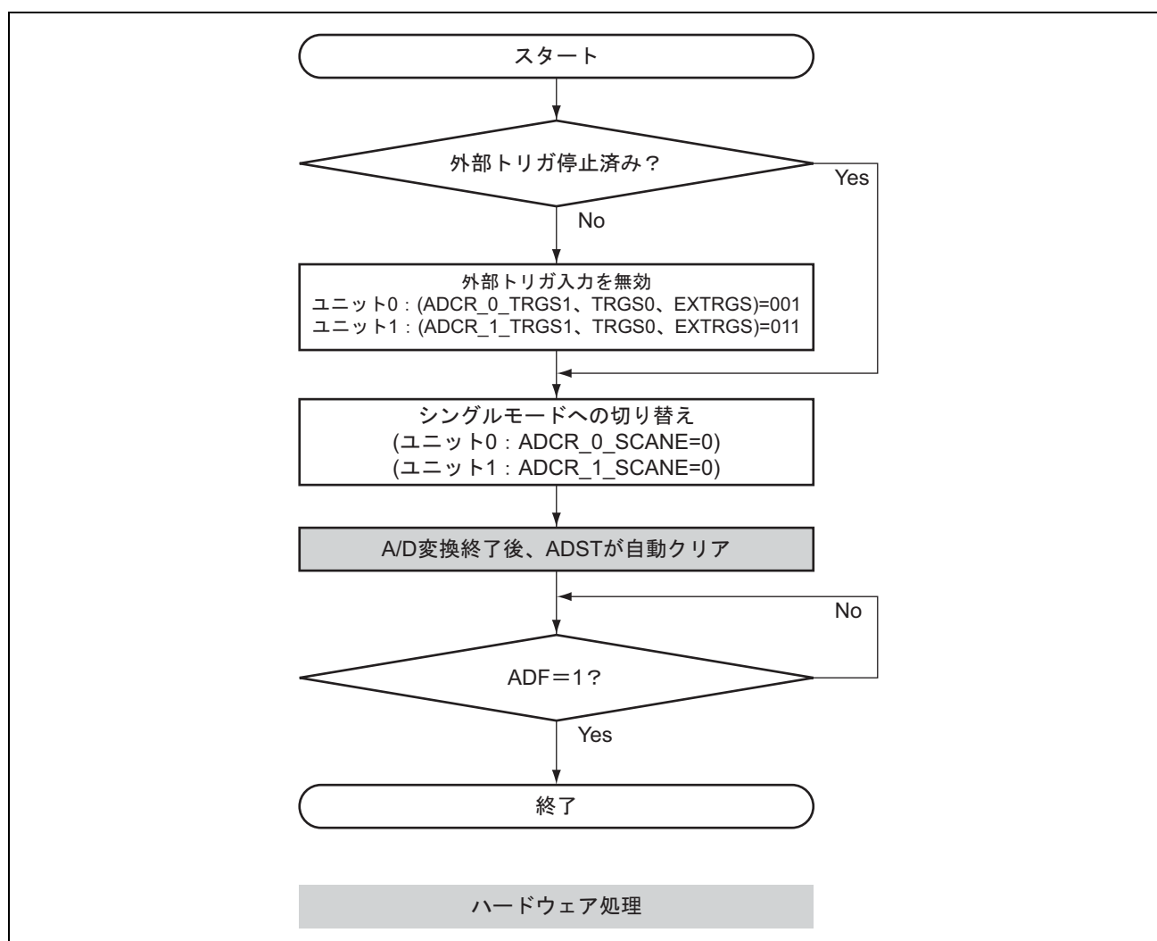
図 19.12 外部トリガによる連続スキャンモード
