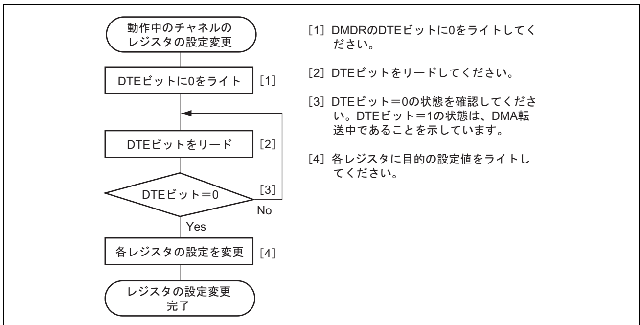
図 10.21 動作中のチャンネルのレジスタ設定を変更するときの手順
