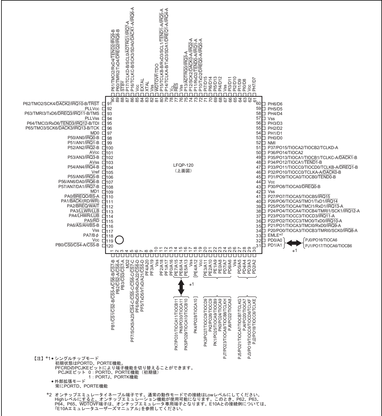
図 1.3 ピン配置図 (LQFP-120 : H8SX/1635 グループ、H8SX/1635L グループ)
