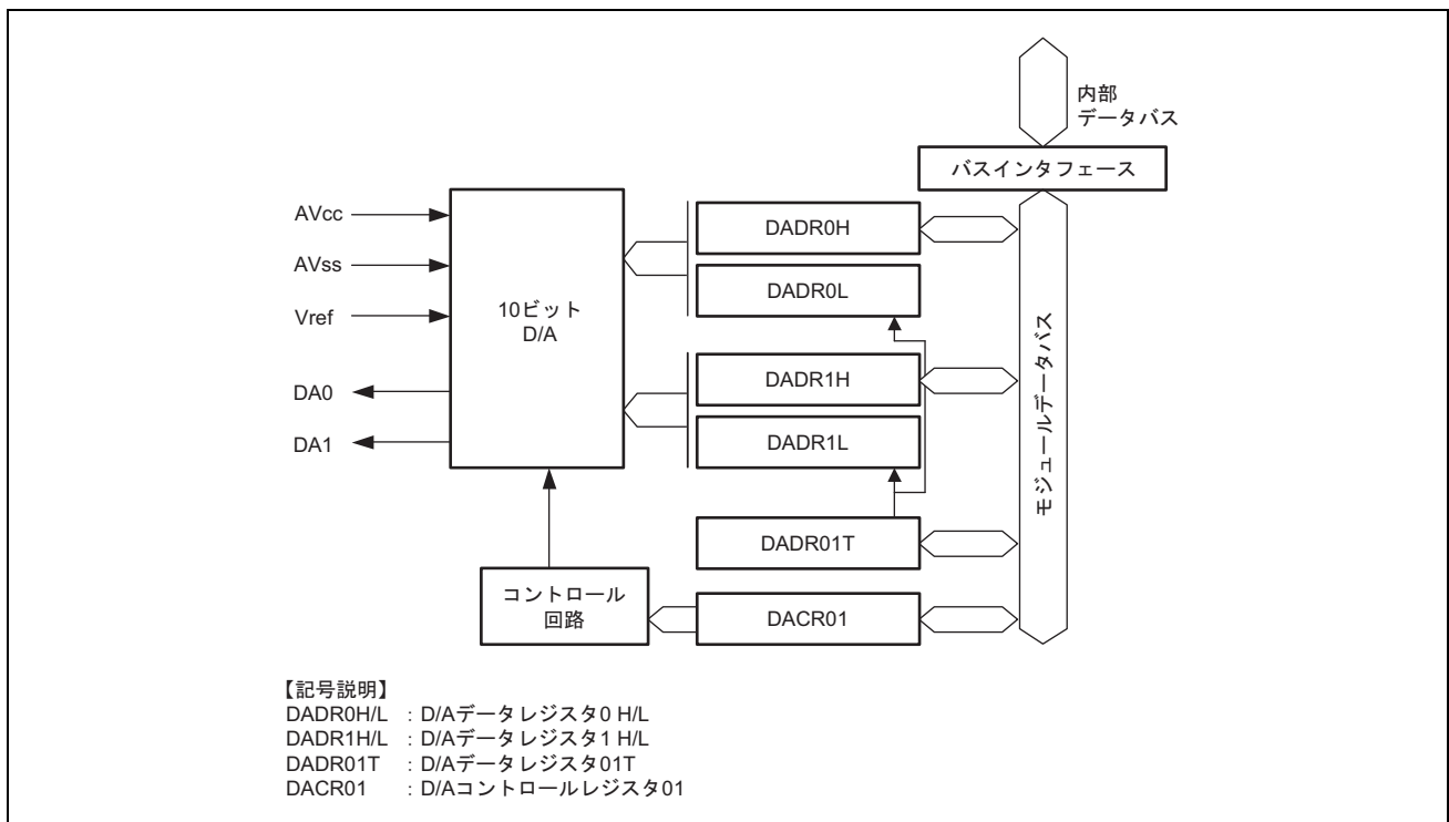
図 20.1 10ビット D/A 変換器のブロック図
