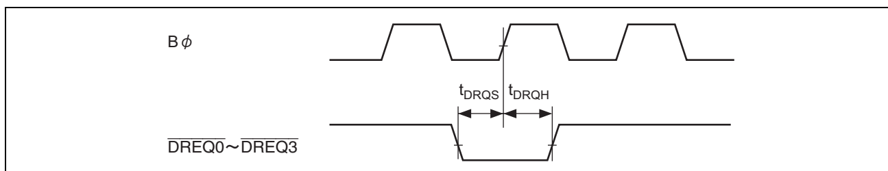
図 27.21 DMAC、 \overline{DREQ} 入力タイミング
