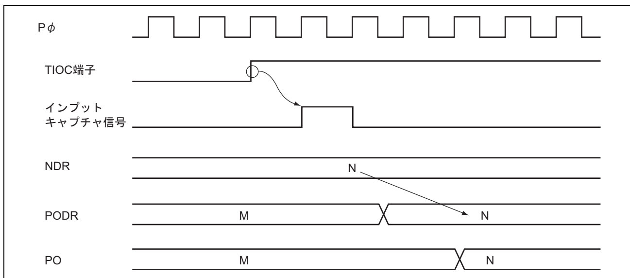
図 14.14 インพุットキャプチャによるパルス出力例
