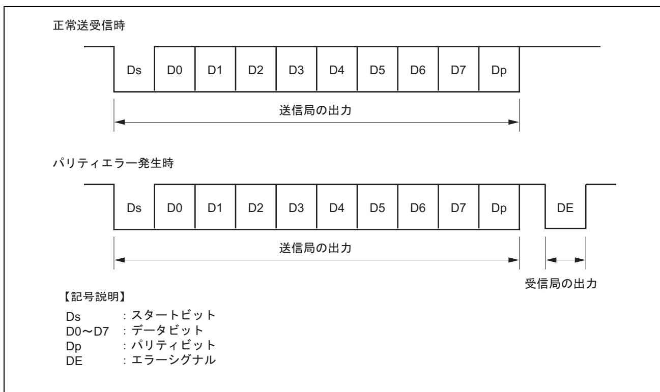
図 17.25 通常のスマートカードインタフェースのデータフォーマット
