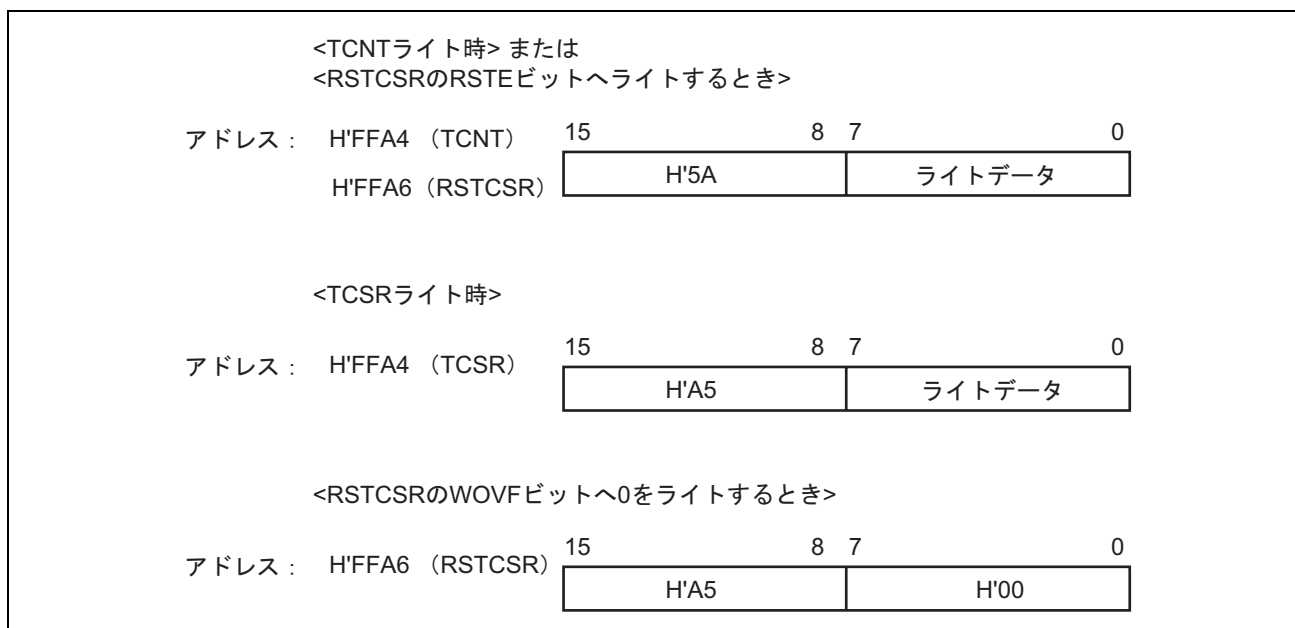
図 16.4 TCNT、TCSR、RSTCSR へのライト
