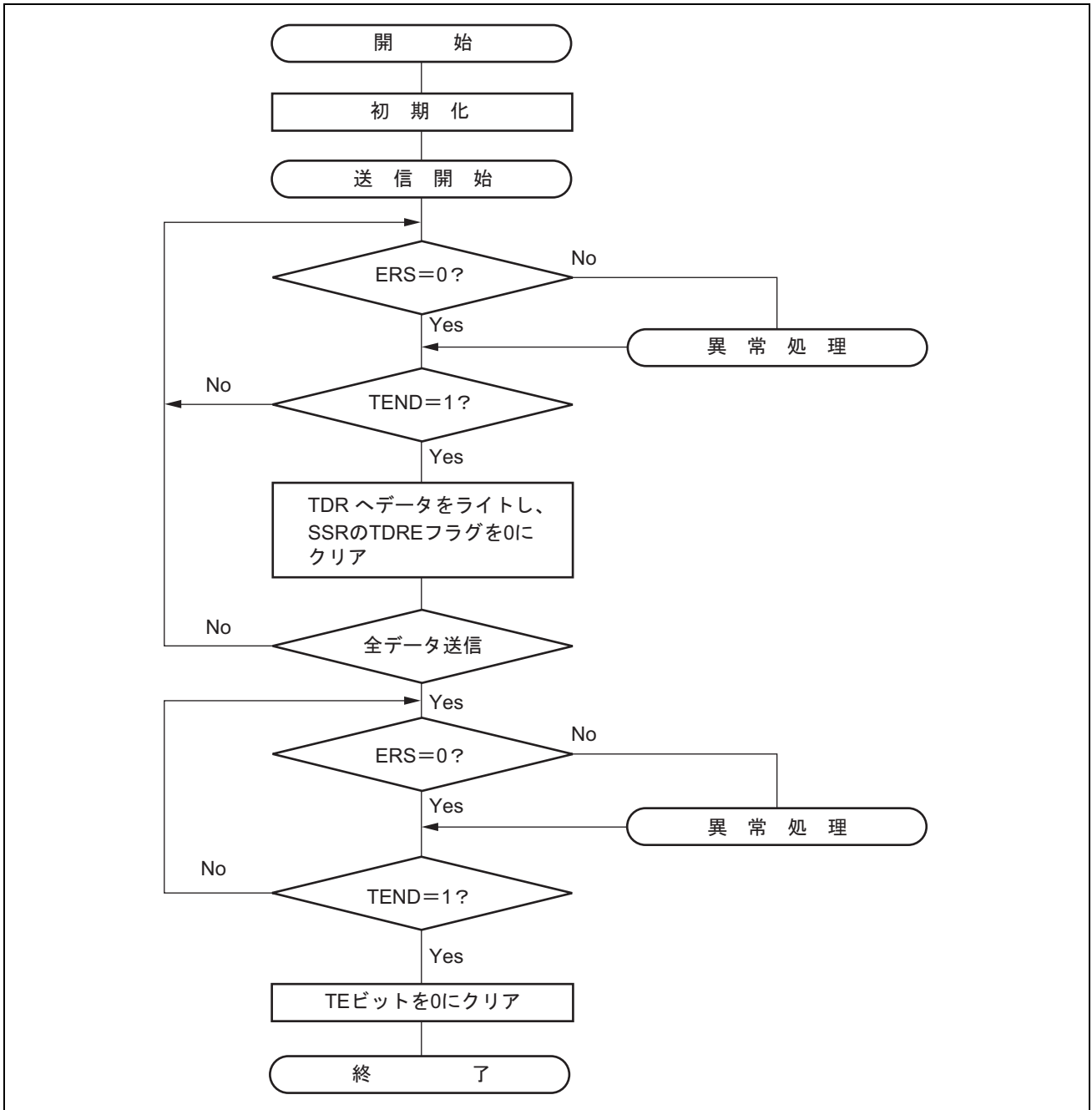
図 17.31 送信処理フローの例
