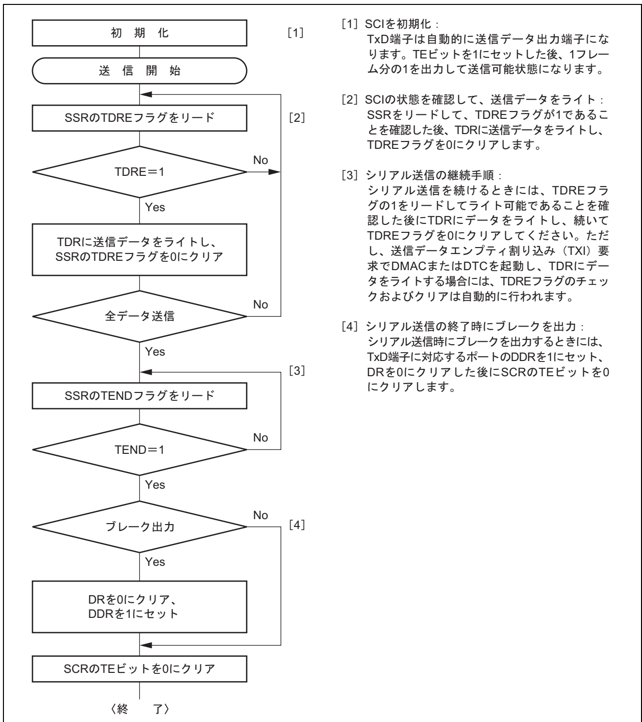
図 17.10 シリアル送信のフローチャートの例
