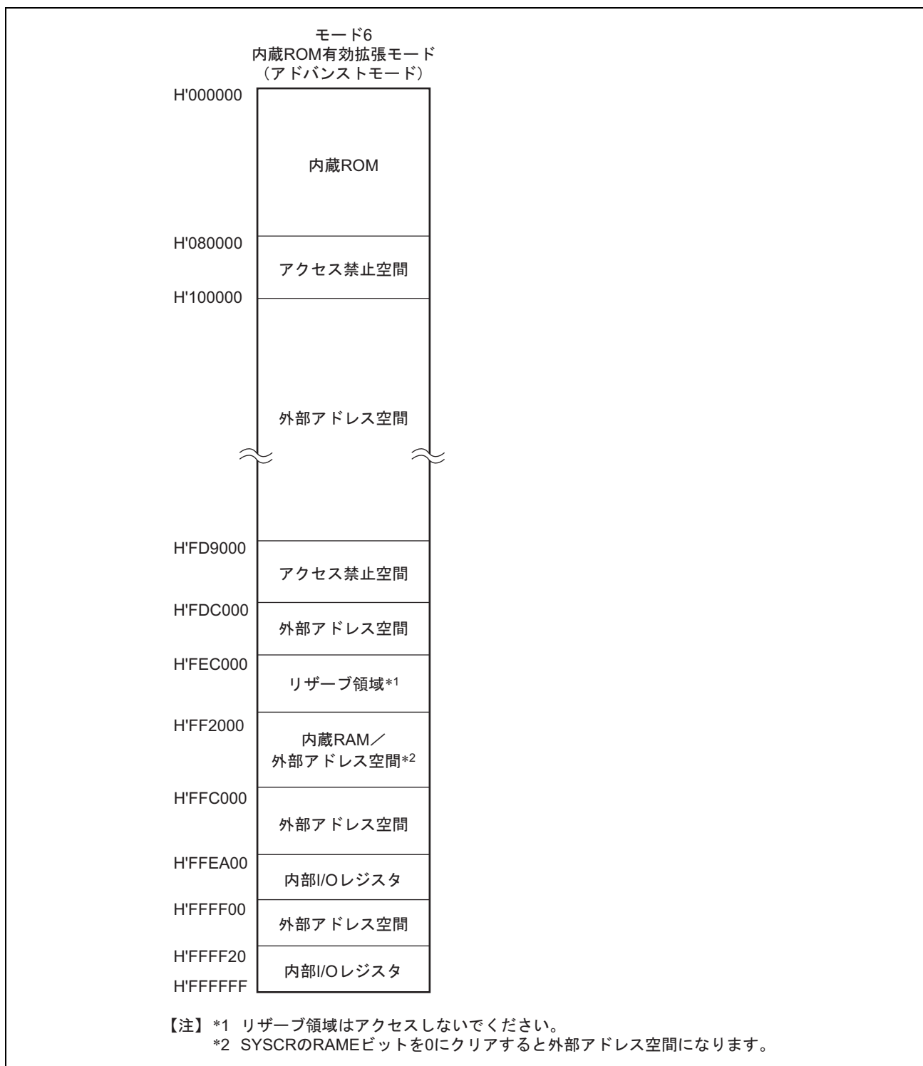
図 3.1 H8SX/1635、H8SX/1635L の各動作モードのアドレスマップ (2)
