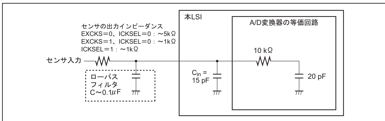
図 19.13 アナログ入力回路の例
