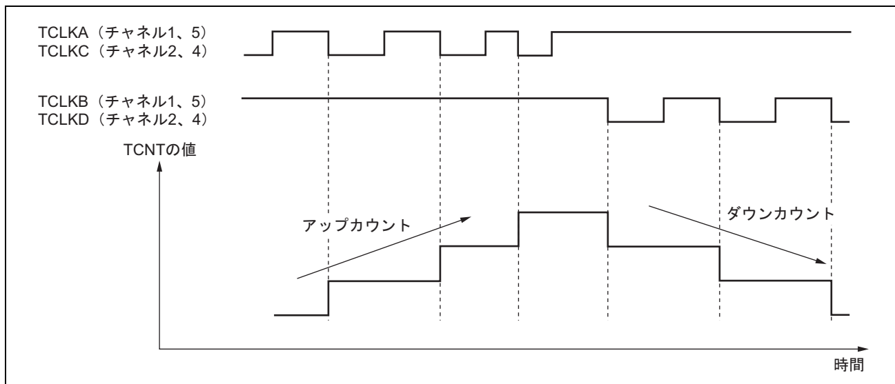
図 13.28 位相計数モード3の動作例
