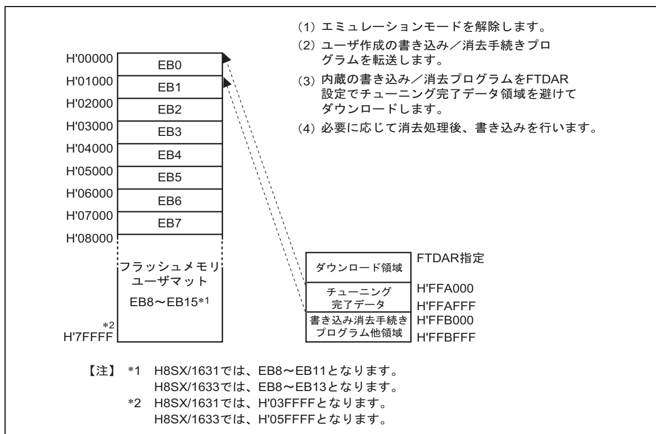
図 22.19 チューニング終了データの書き込み (H8SX/1635)
