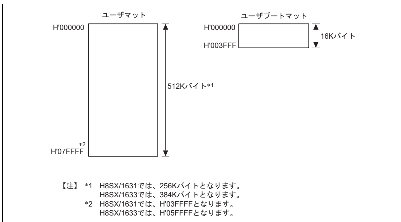
図 22.3 メモリマツト構成 (H8SX/1635)
