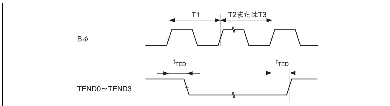
図 27.22 DMAC、 \overline{TEND} 出力タイミング
