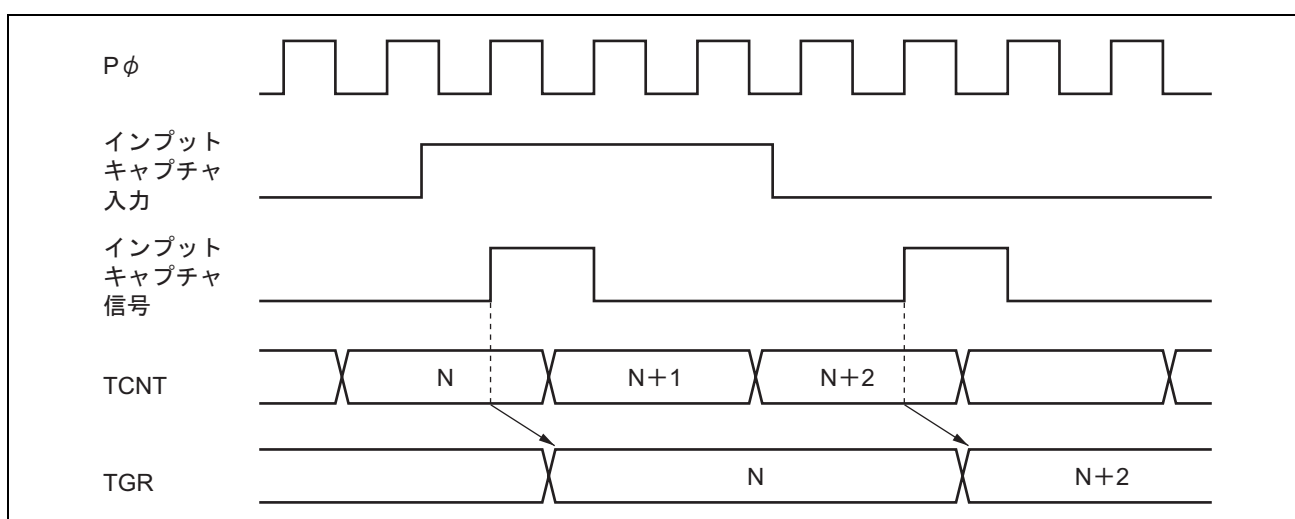
図 13.34 インพุットキャプチャ入力信号タイミング
