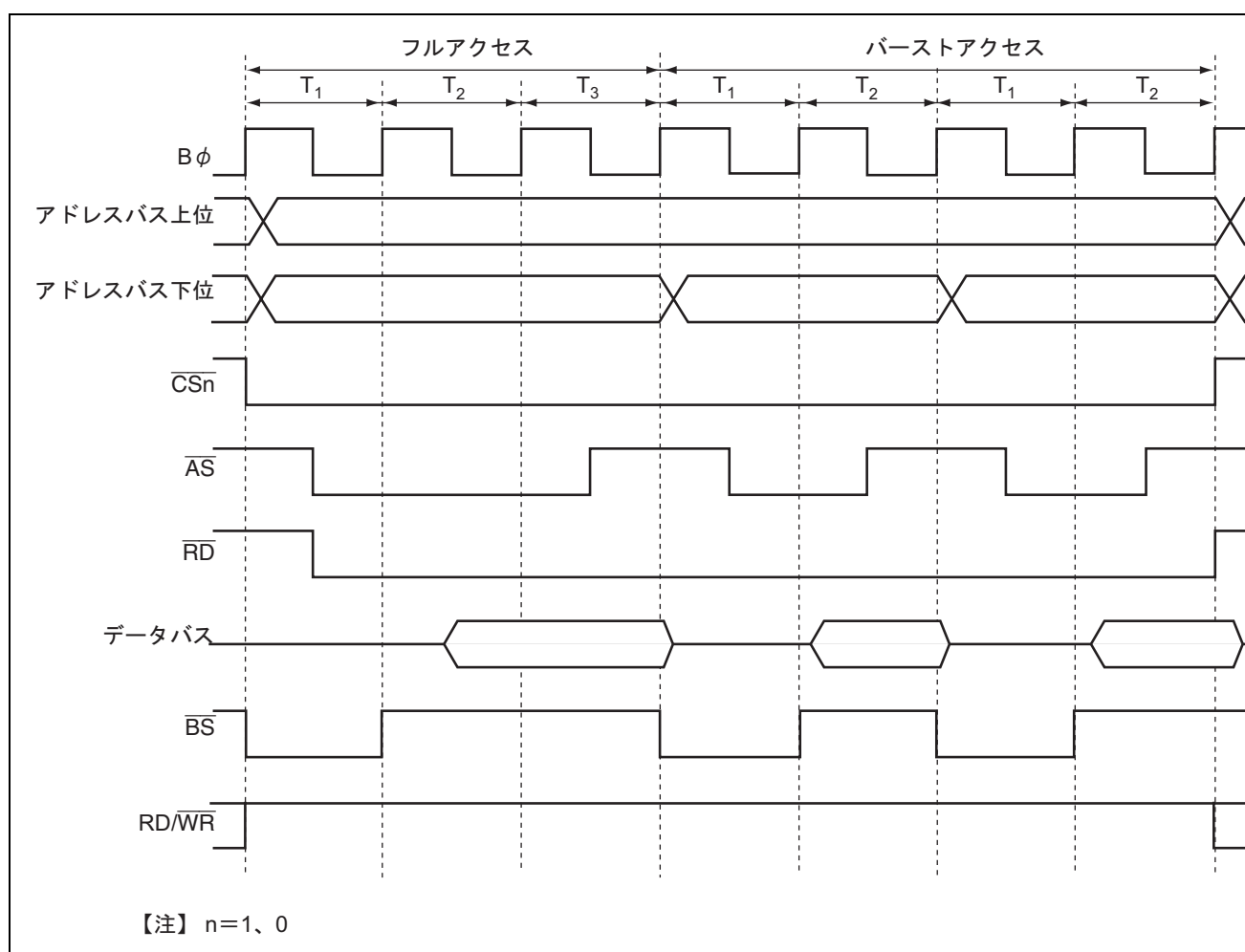
図 9.28 バースト ROM アクセスタイミング例 (ASTn=1、バーストサイクル 2 ステート)
