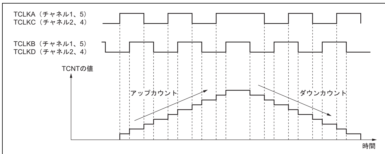
図 13.26 位相計数モード 1 の動作例
