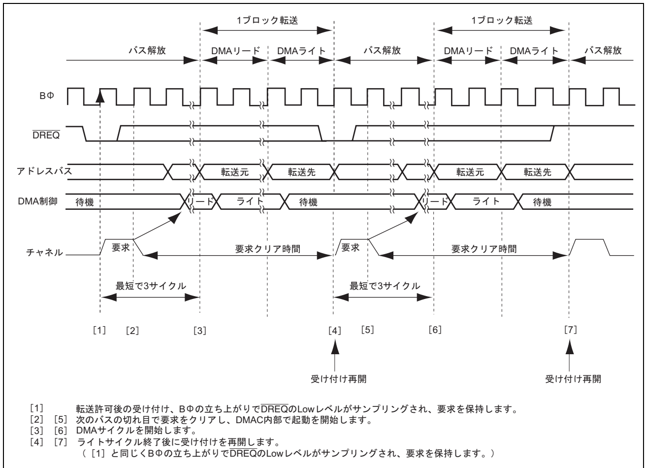
図 10.32 DREQ レベル起動時のブロック転送モードの転送例
