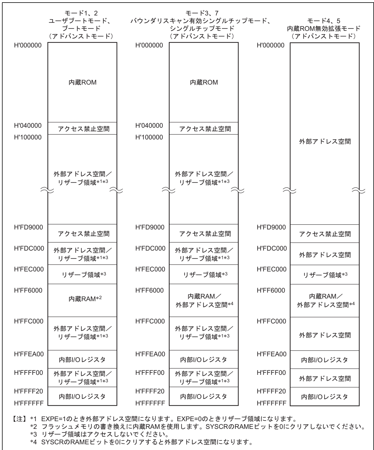
図 3.3 H8SX/1631、H8SX/1631L の各動作モードのアドレスマップ (1)
