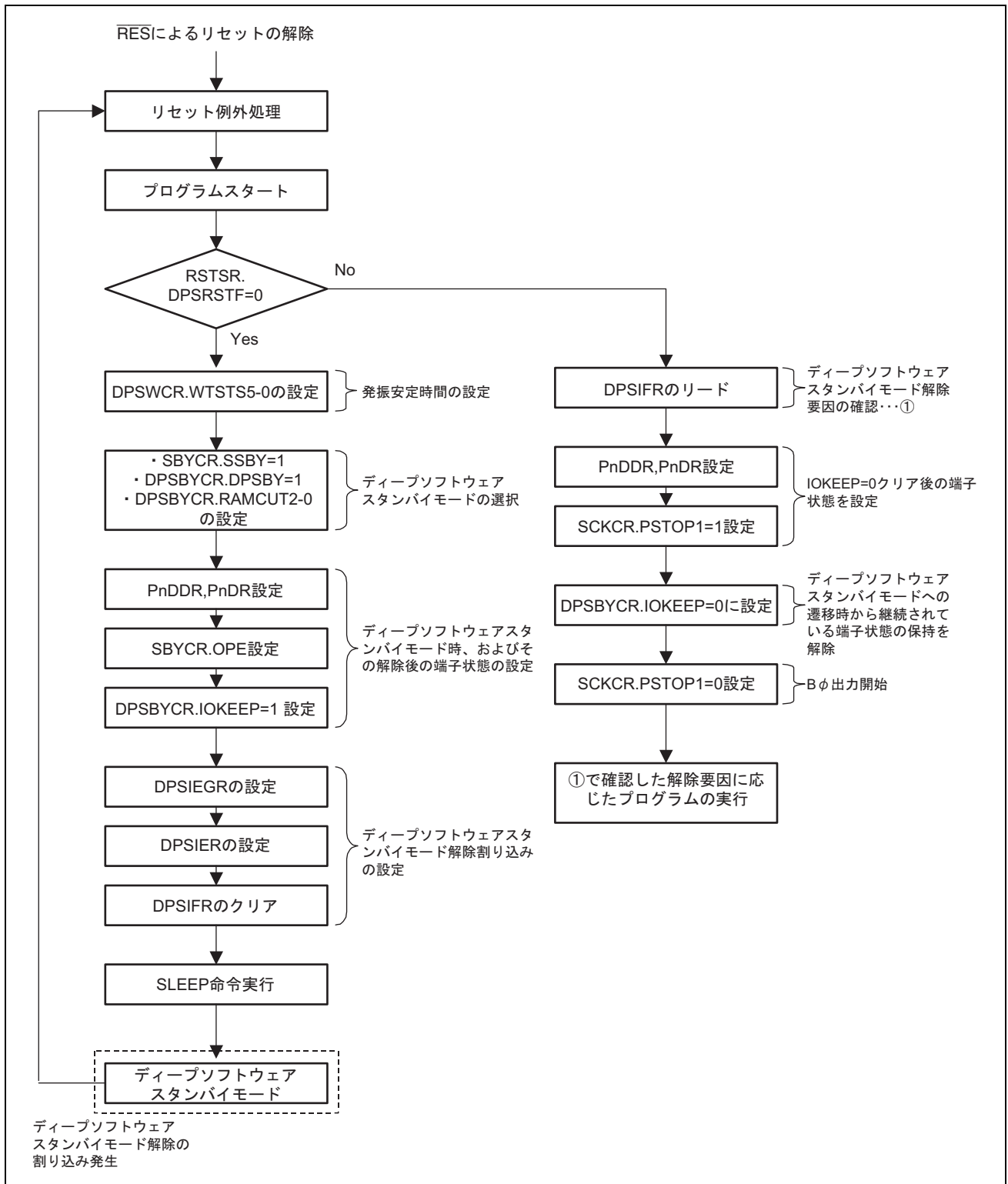
図 25.7 ディープリフトウェアスタンバイモードのフローチャート例
