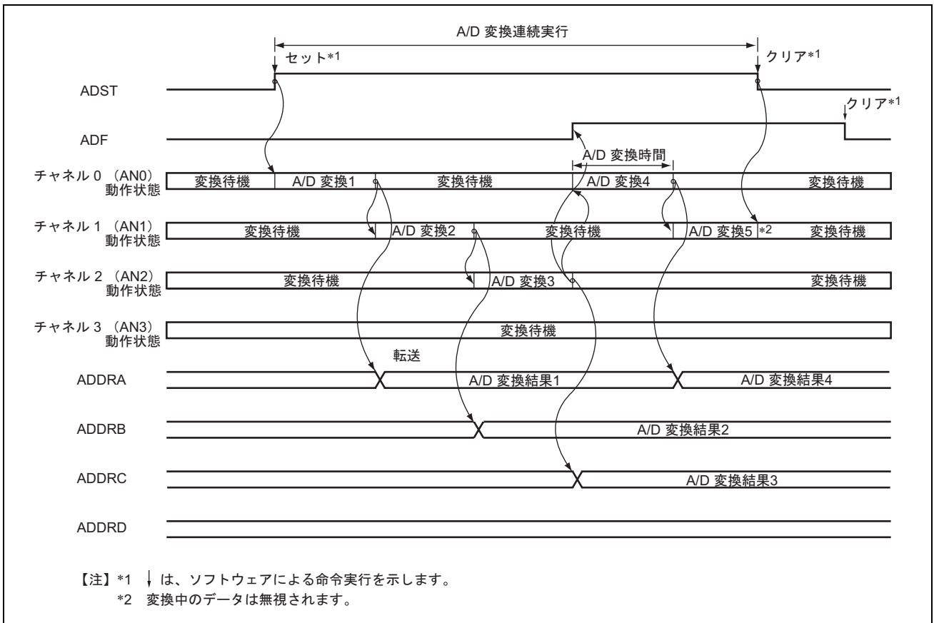
図 19.4 A/D 変換器の動作例 (連続スキャンモード、AN0~AN2 の 3 チャンネル選択時)
