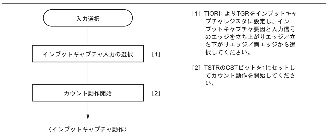
図 13.9 インพุットキャプチャ動作の設定例
