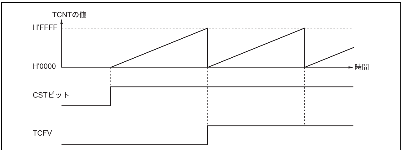
図 13.4 フリーランニングカウンタの動作
