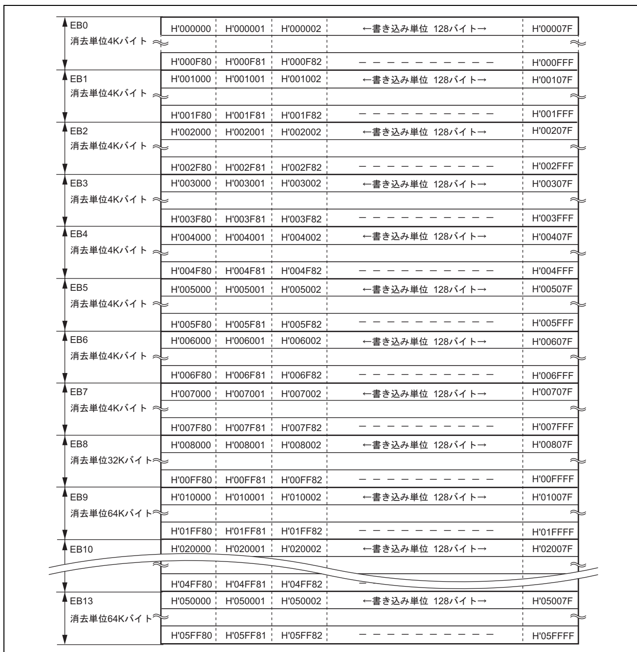
図 22.4 (2) H8SX/1633 のユーザマットのブロック構成
