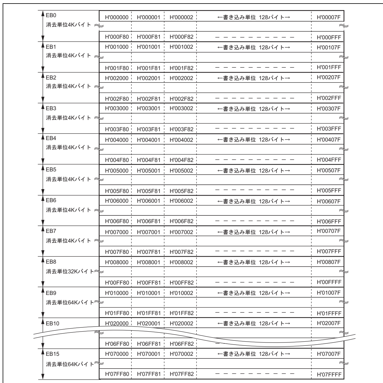
図 22.4 (3) H8SX/1635 のユーザマットのブロック構成
