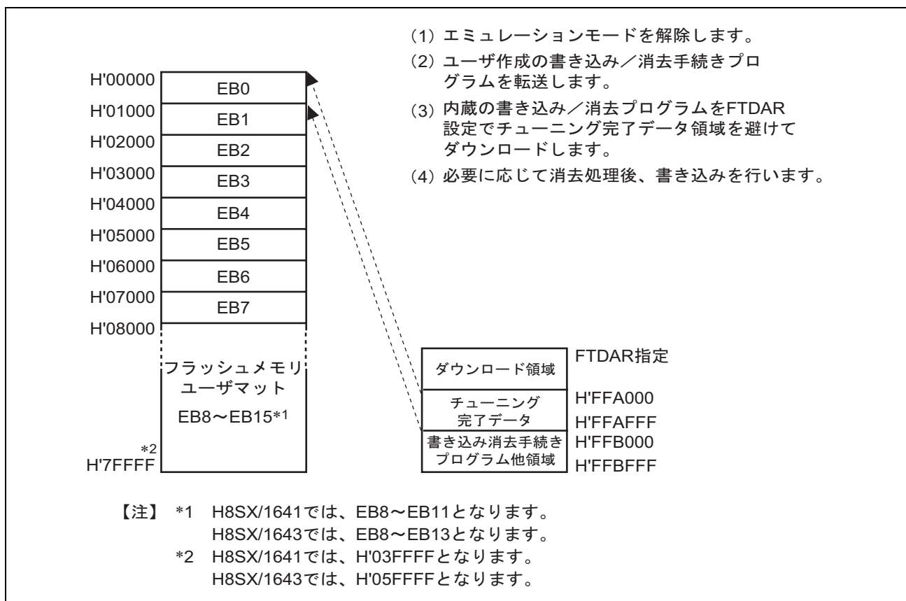
図 22.19 チューニング終了データの書き込み (H8SX/1645)
