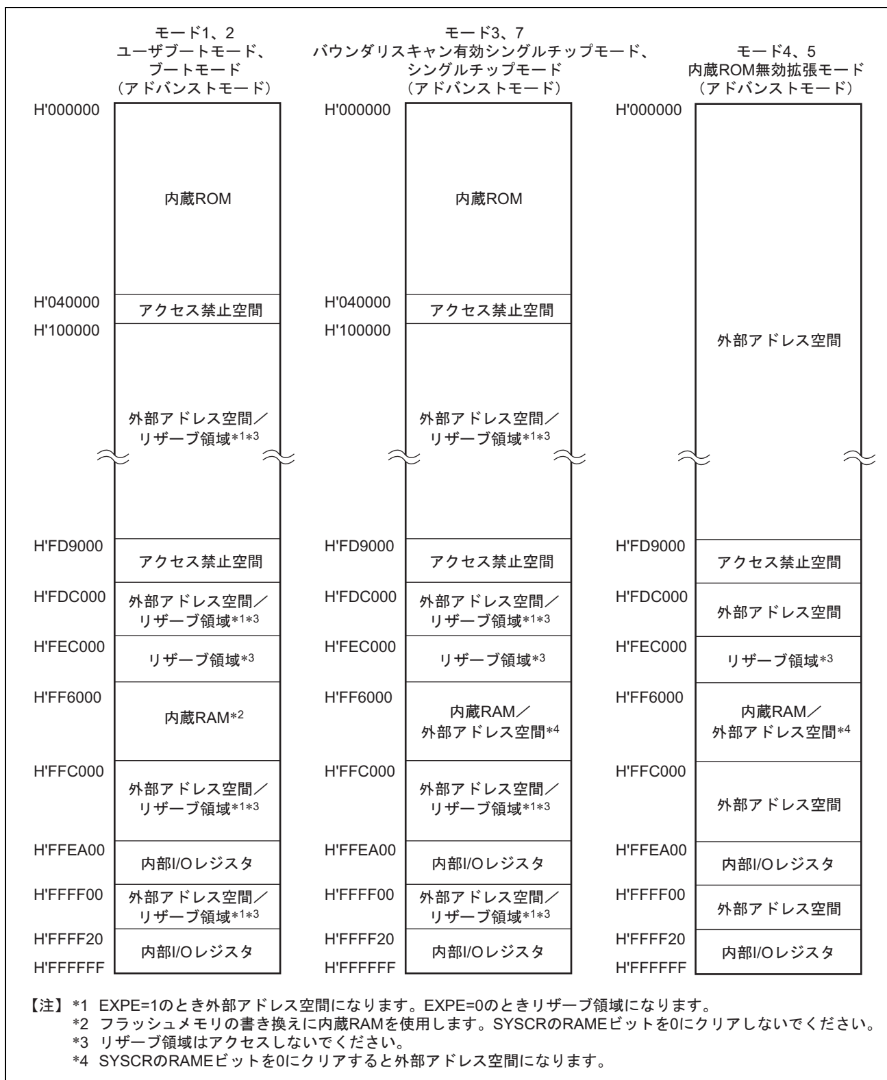
図 3.3 H8SX/1641、H8SX/1641L の各動作モードのアドレスマップ (1)
