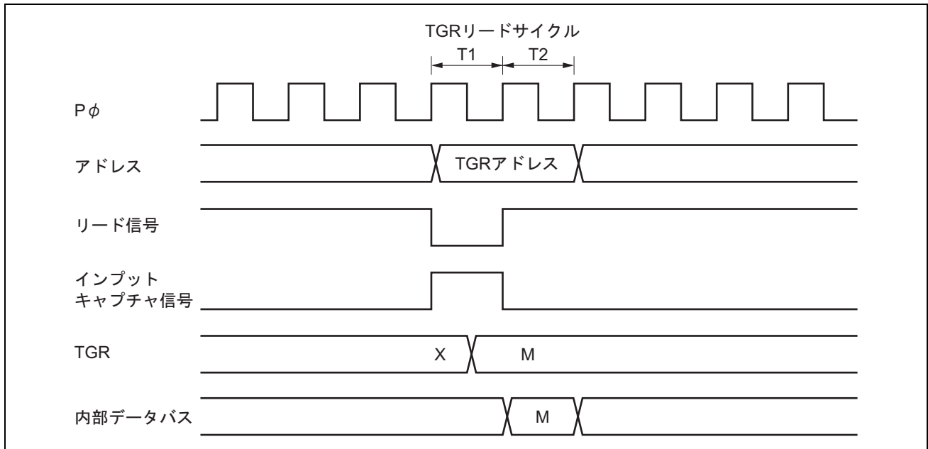
図 13.51 TGRのリードと入力キャプチャの競合
