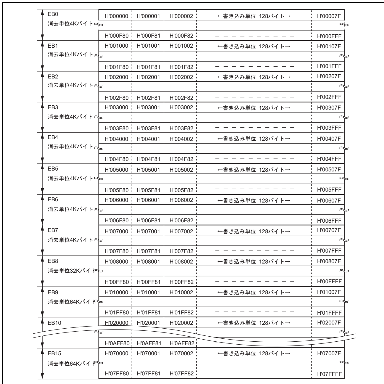
図 22.4 (3) H8SX/1645 のユーザマットのブロック構成
