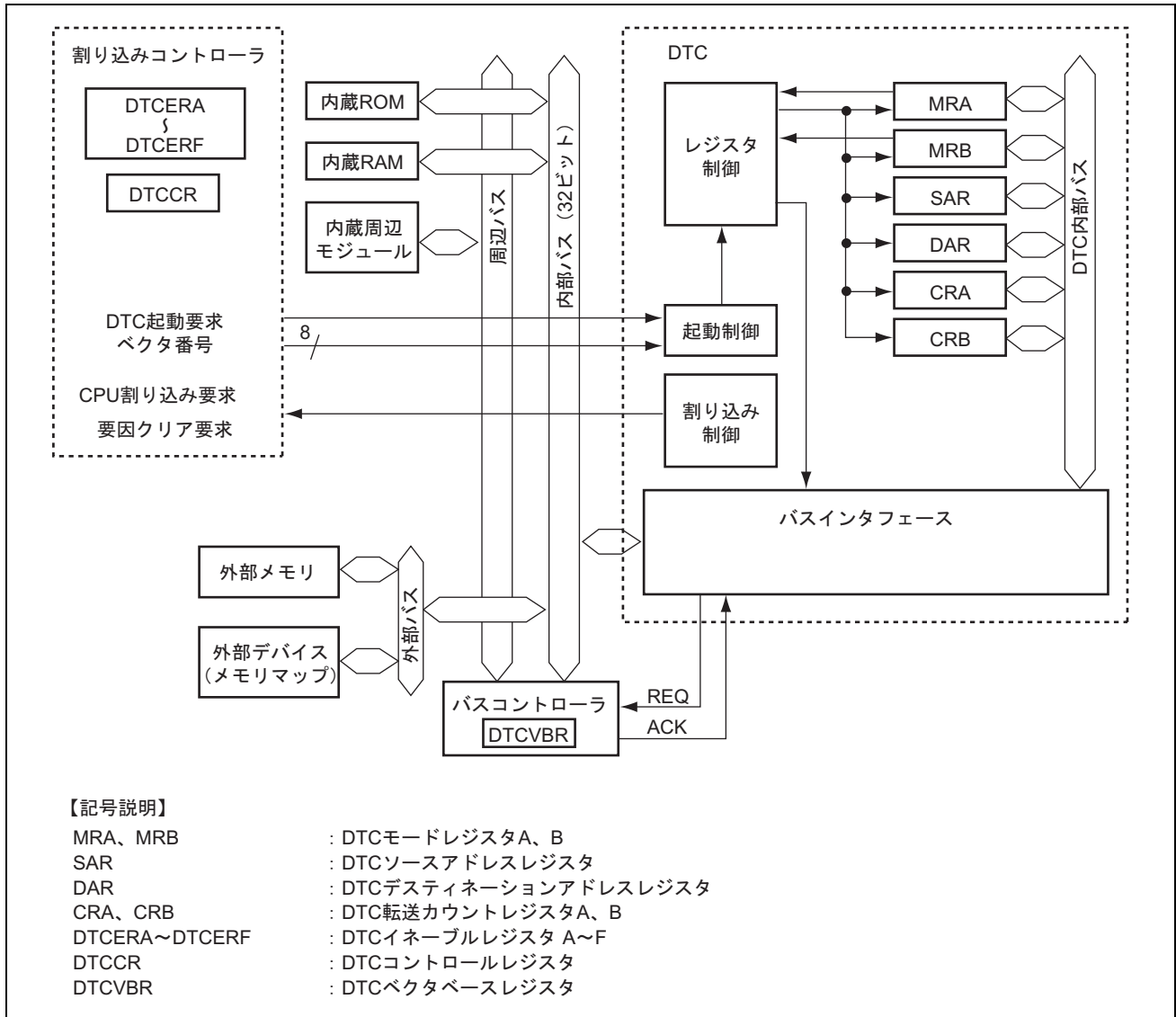
図 11.1 DTC のブロック図
