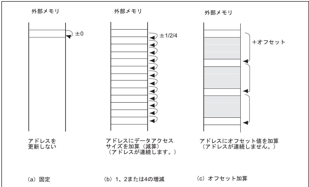
図 10.17 アドレスの更新方法
