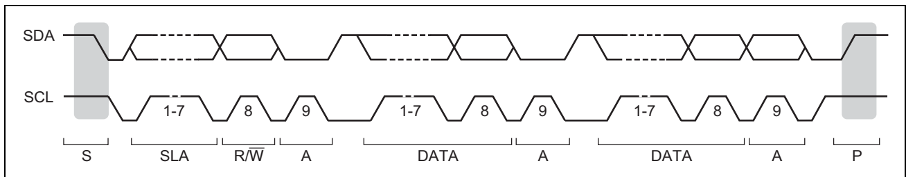
図 18.4 I 2 C バスタイミング
