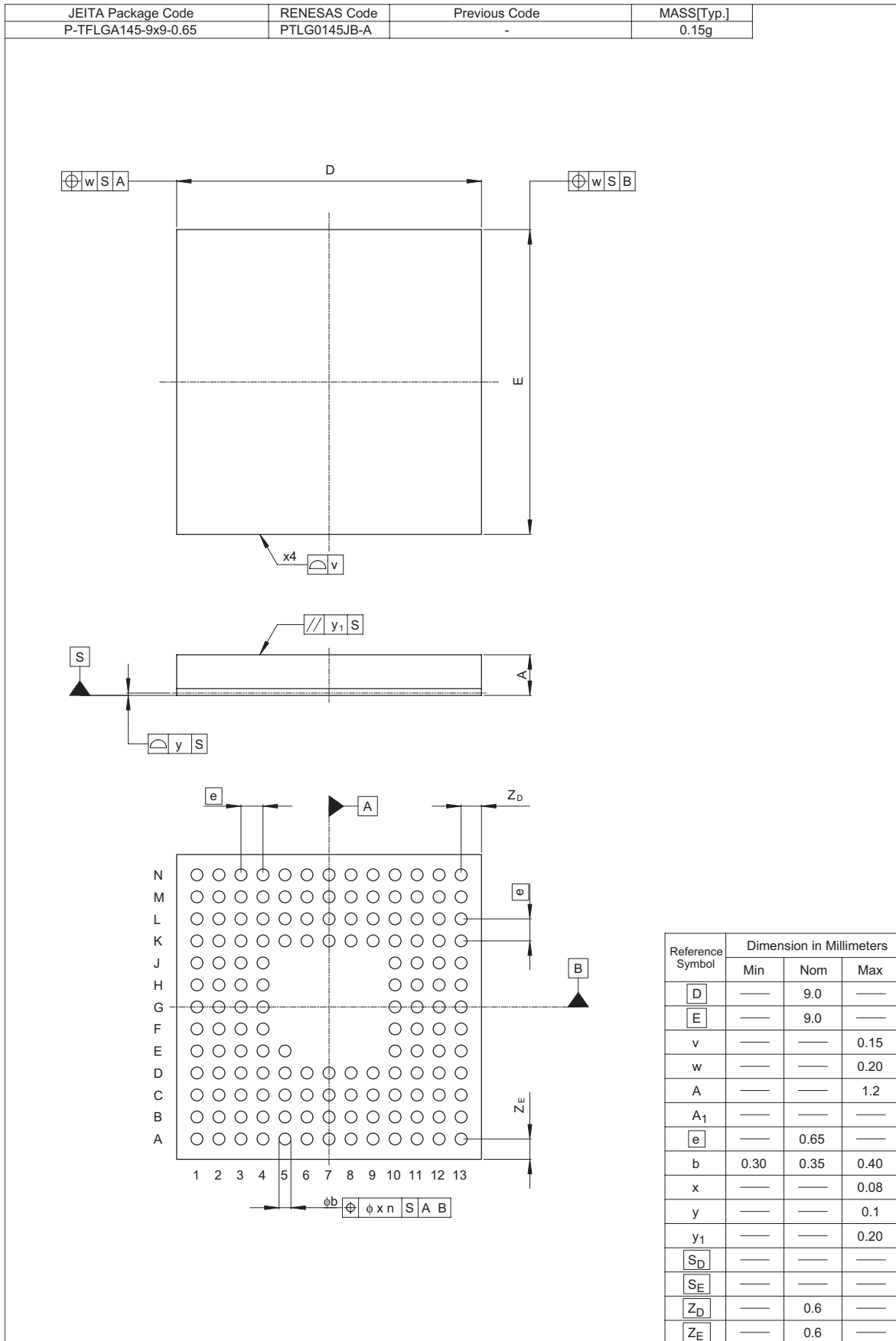
図 C.2 外形寸法図 (TLP-145V)
