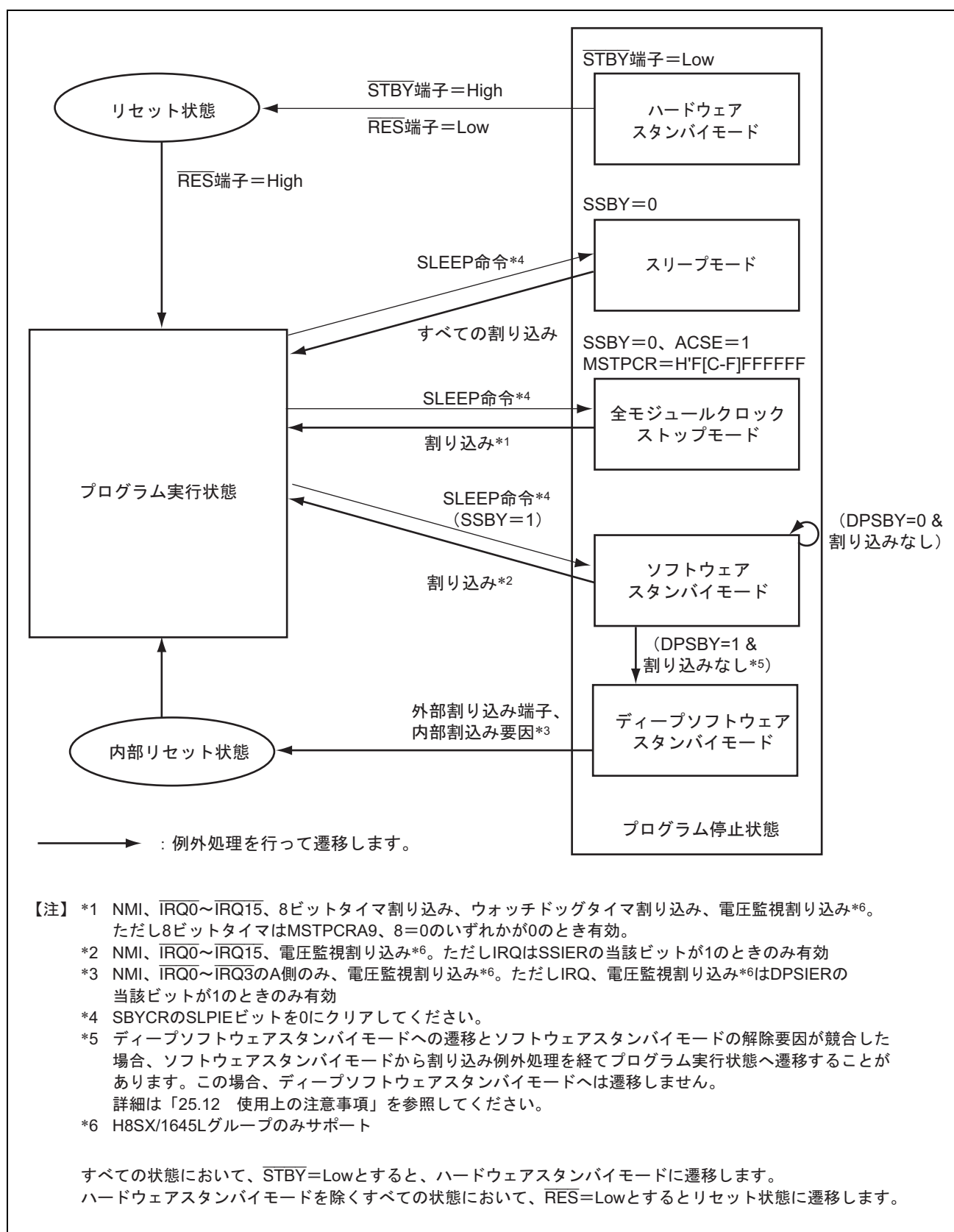
図 25.1 モード遷移 (H8SX/1645、H8SX/1645L グループ)
