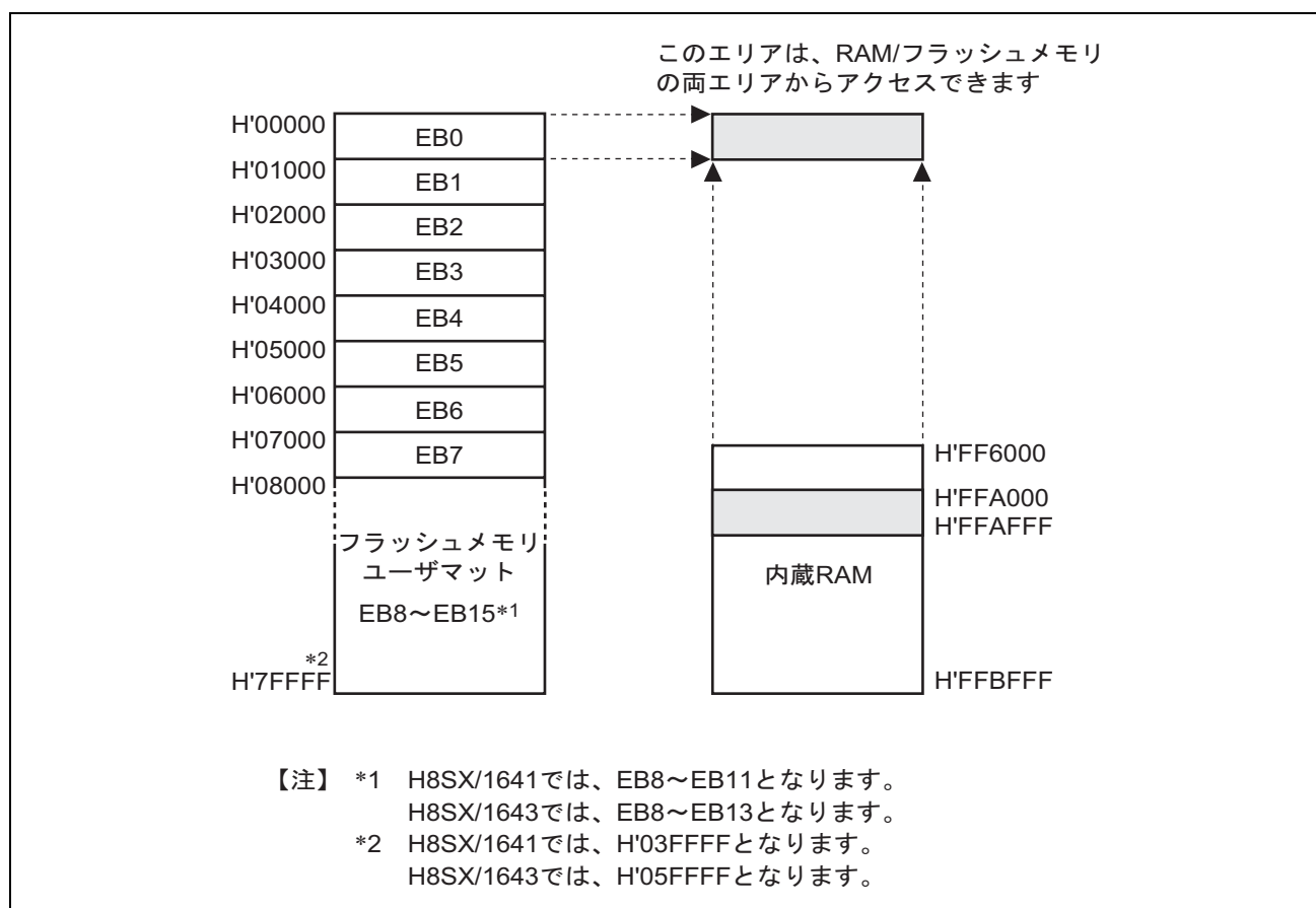
図 22.18 RAM のオーバーラップ動作例 (H8SX/1645)
