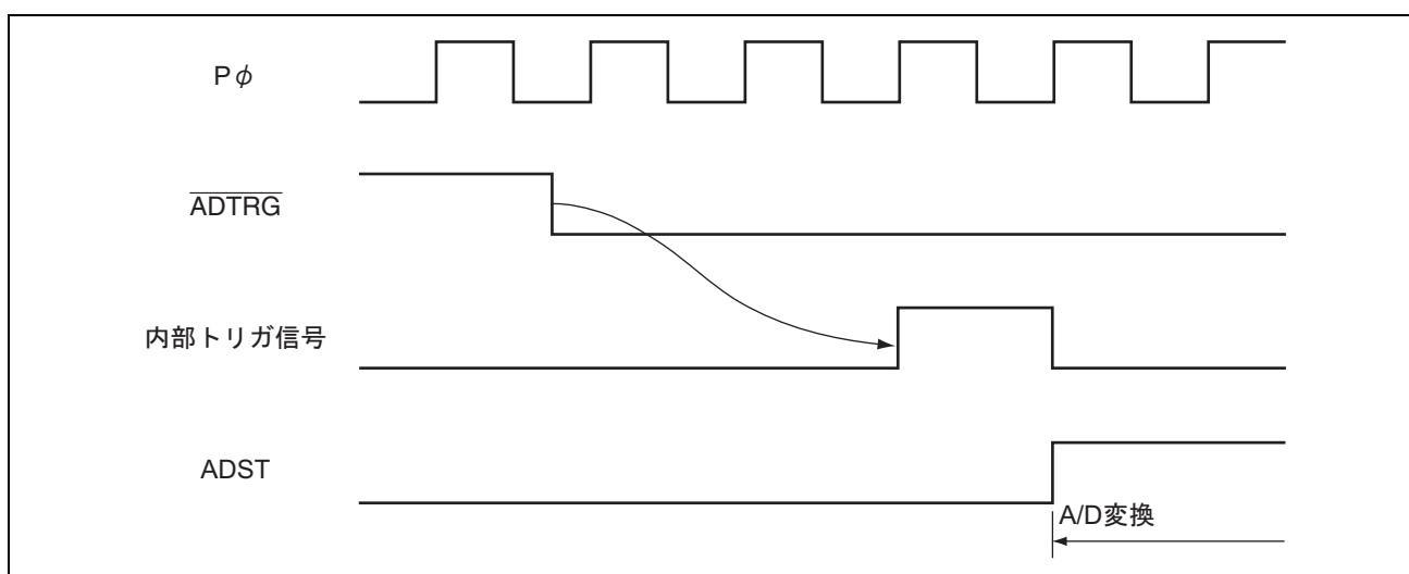
図 19.8 外部トリガ入力タイミング (TRGS1、TRGS0、EXTRGS≠B'111)
