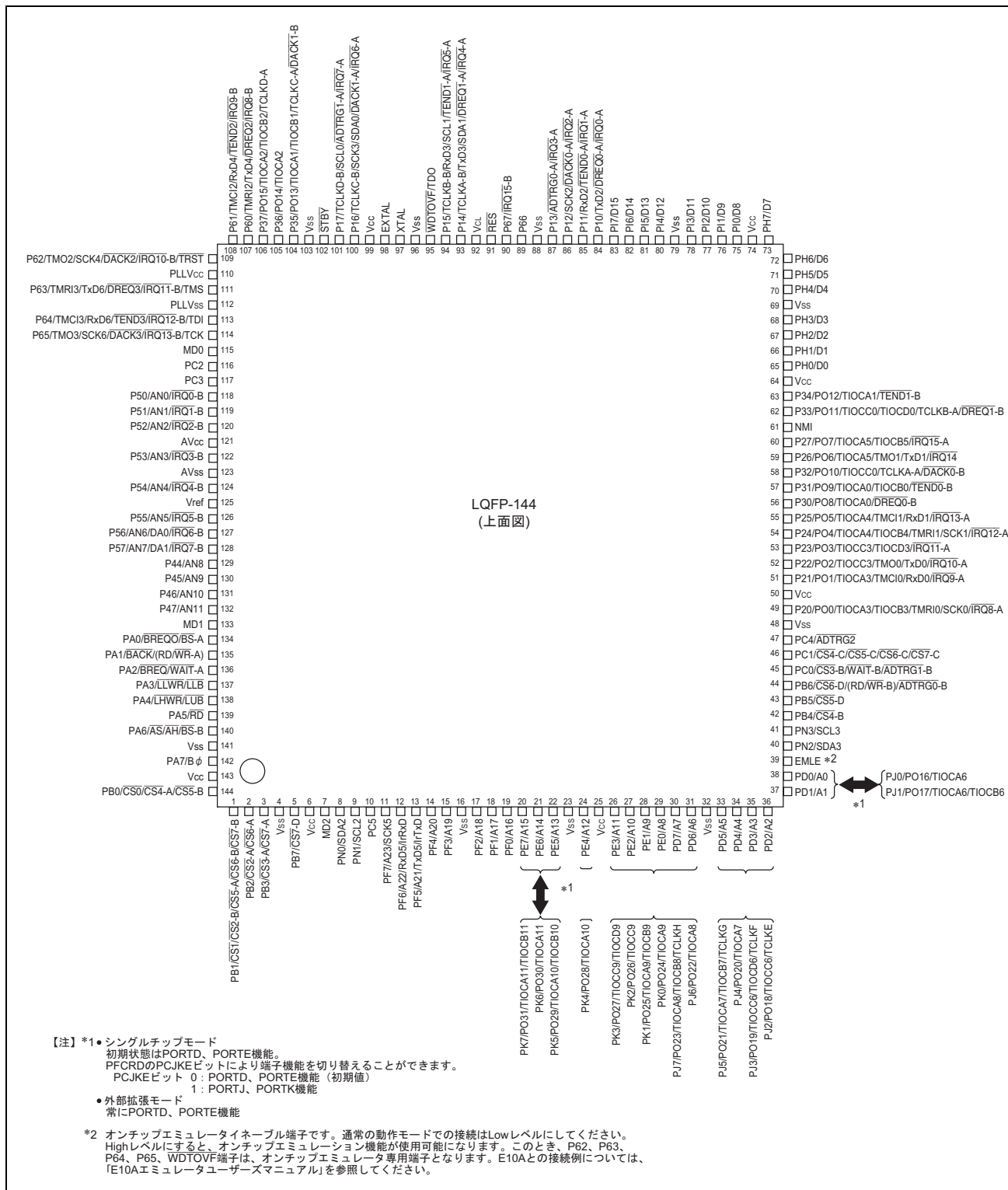
図 1.3 ピン配置図 (LQFP-144:H8SX/1645、H8SX/1645L グループ)
