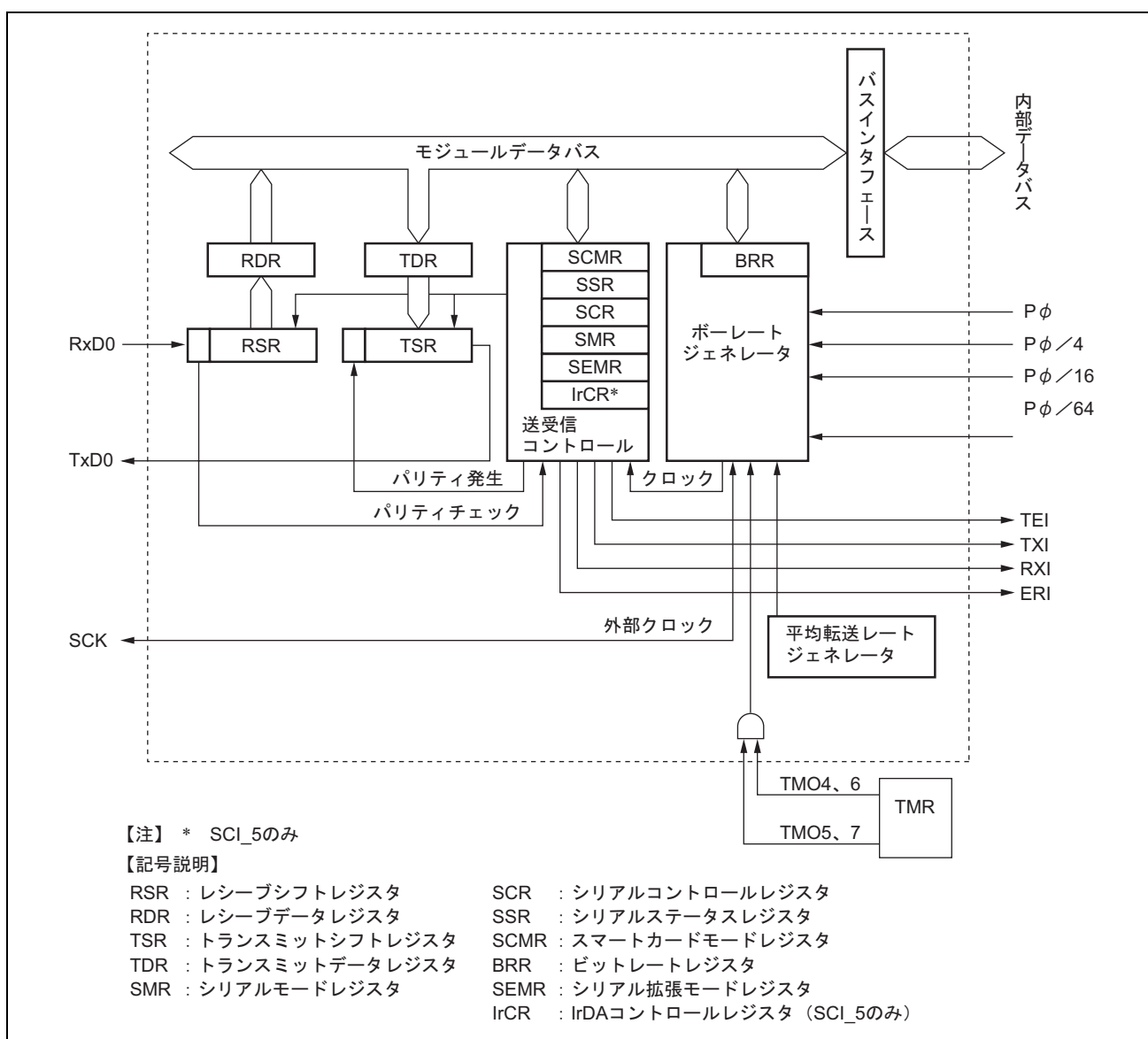
図 17.2 SCI_5、6 のブロック図
