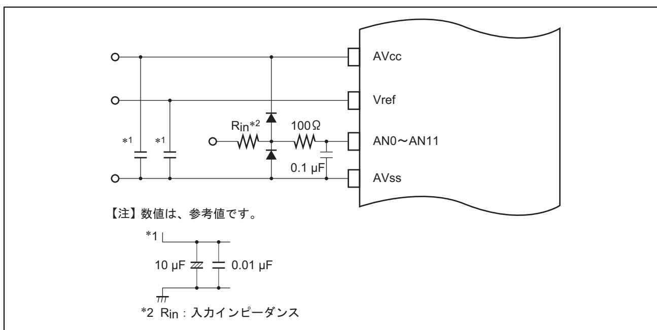
図 19.22 アナログ入力保護回路の例
