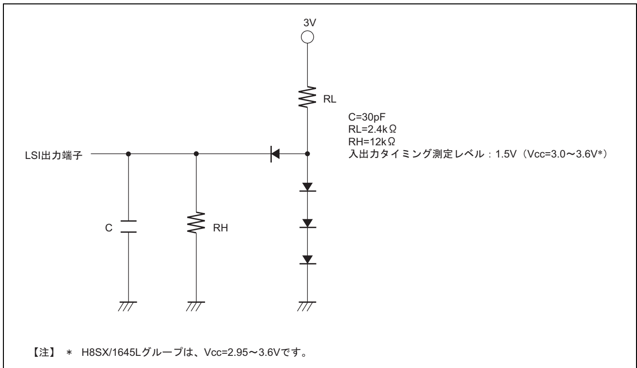
図 27.1 出力負荷回路
