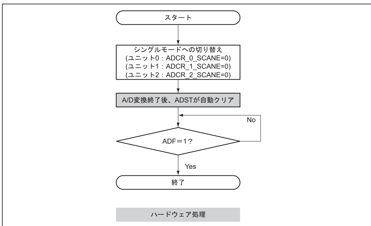
図 19.12 ソフトウェア起動による連続スキャンモード停止方法
