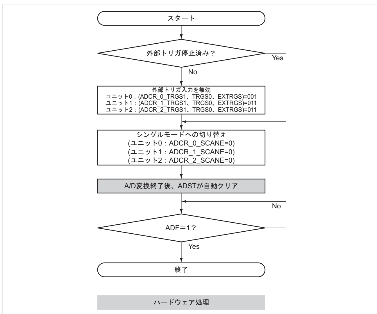
図 19.13 外部トリガによる連続スキャンモード
