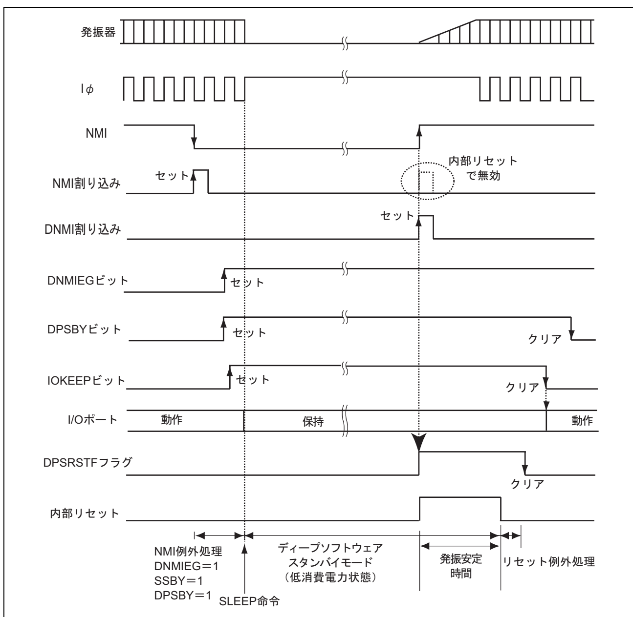
図 25.4 ディープソフトウェアスタンバイモードの応用例 (IOKEEP ビットが 1 のとき)
