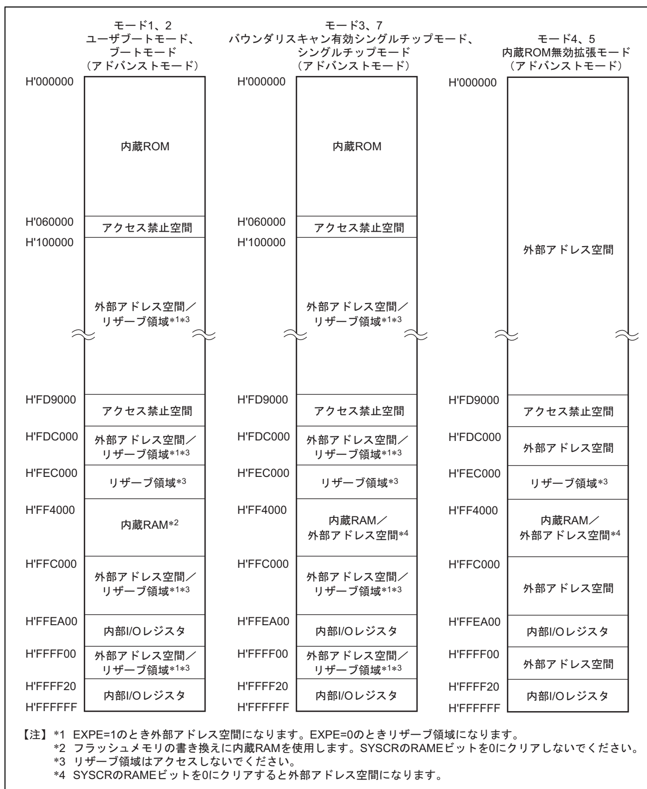
図 3.2 H8SX/1643、H8SX/1643L の各動作モードのアドレスマップ (1)
