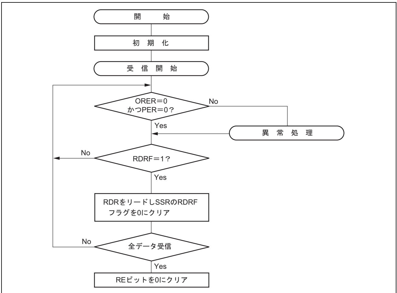
図 17.33 受信フローの例
