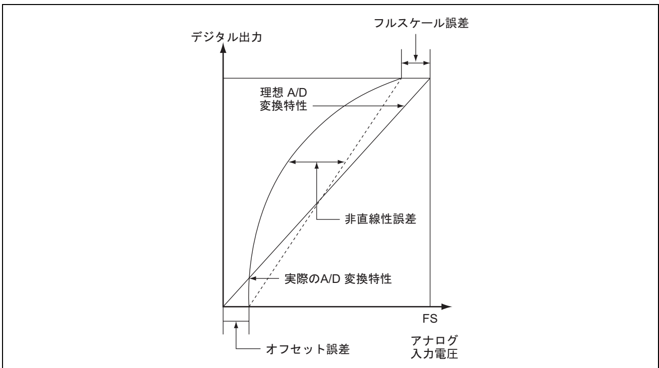
図 19.11 A/D 変換精度の定義
