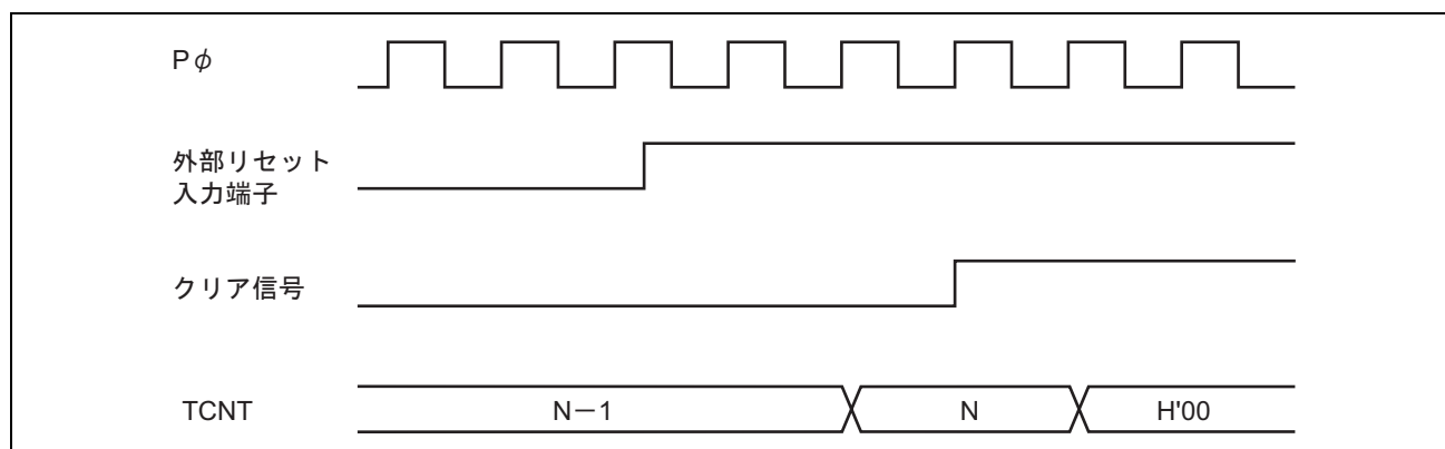
図 15.13 外部リセット入力によるクリアタイミング (ハイレベル)
