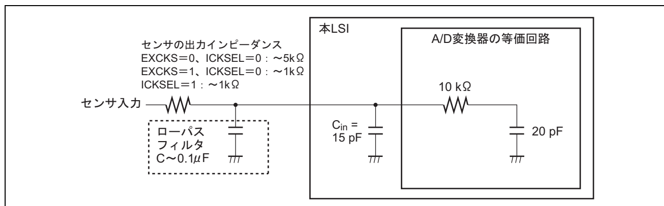
図 19.21 アナログ入力回路の例
