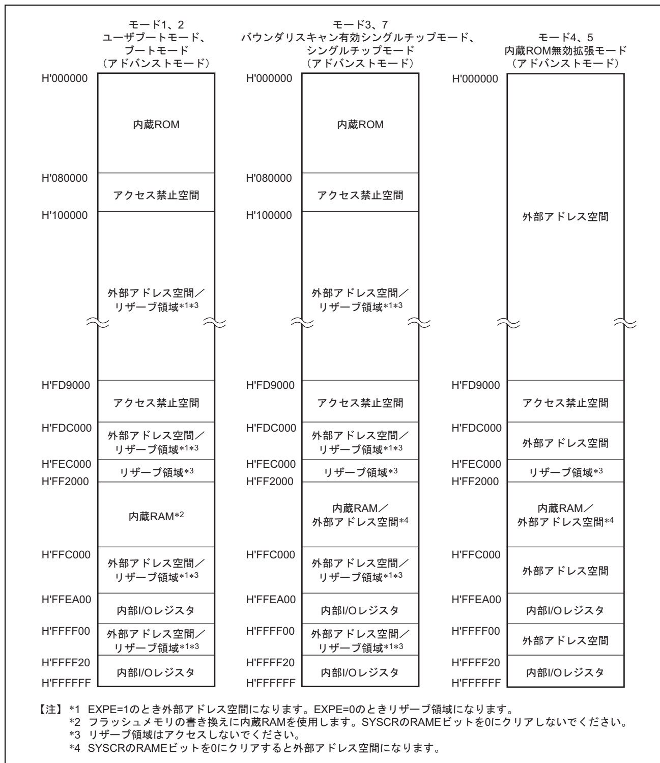
図 3.1 H8SX/1645、H8SX/1645L の各動作モードのアドレスマップ (1)
