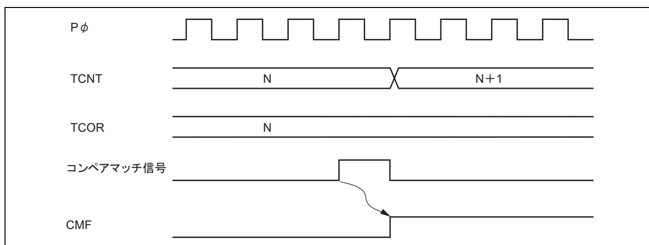
図 15.9 コンペアマッチ時の CMF フラグのセットタイミング
