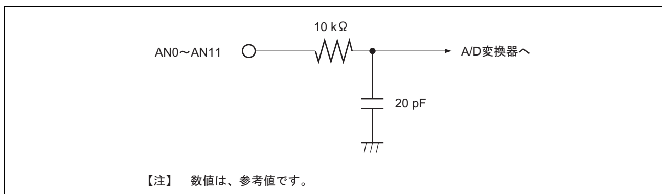
図 19.23 アナログ入力端子等価回路
