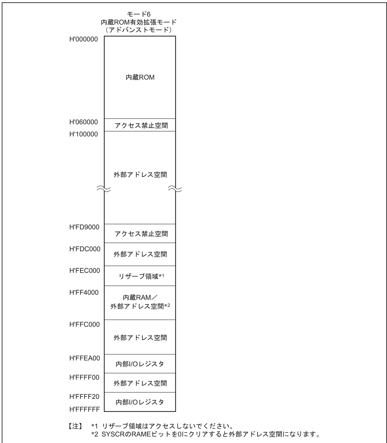
図 3.2 H8SX/1643、H8SX/1643L の各動作モードのアドレスマップ (2)
