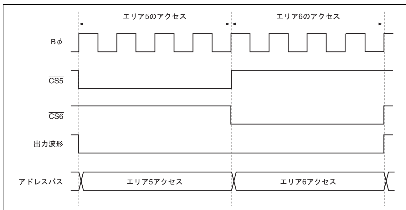
図 9.9 \overline{CS} を同一端子に出力したときのタイミング
