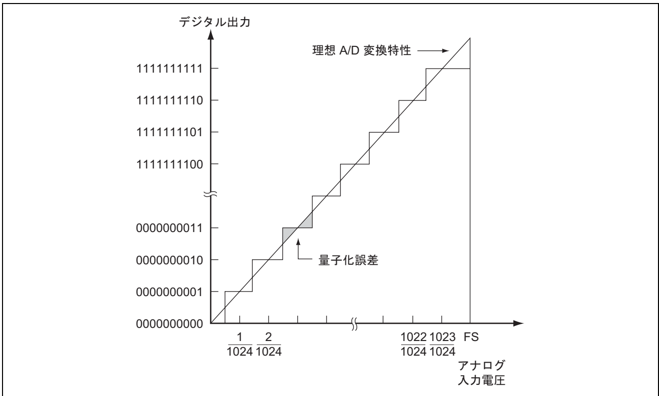
図 19.10 A/D 変換精度の定義
