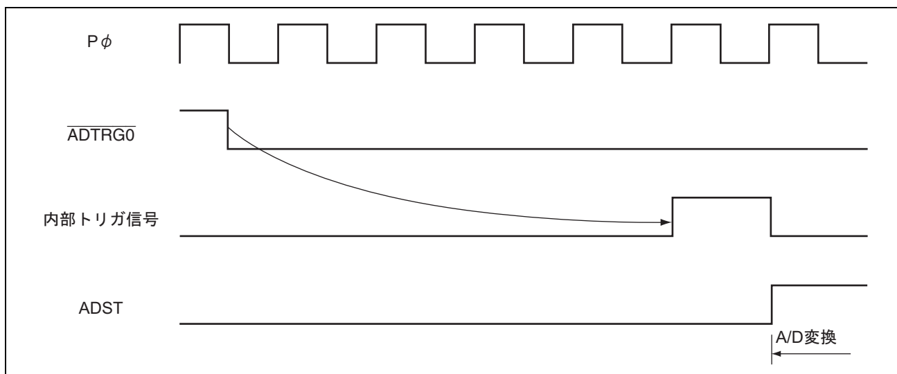
図 19.9 外部トリガ入力タイミング (ユニット同時起動時 : TRGS1、TRGS0、EXTRGS=B'111)
