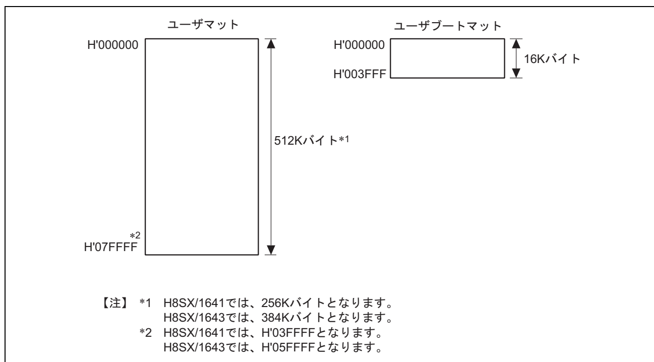
図 22.3 メモリマツト構成 (H8SX/1645)
