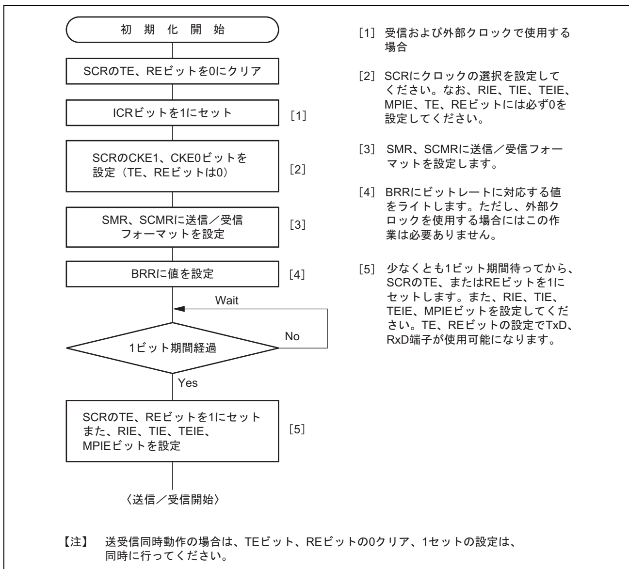
図 17.18 SCI の初期化フローチャートの例
