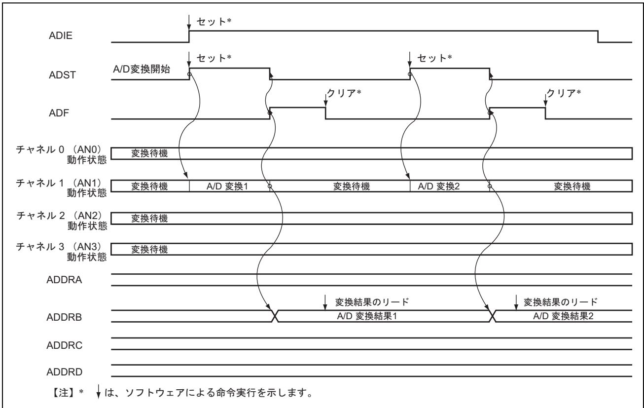
図 19.4 A/D 変換器の動作例 (シングルモード、チャンネル 1 選択時)
