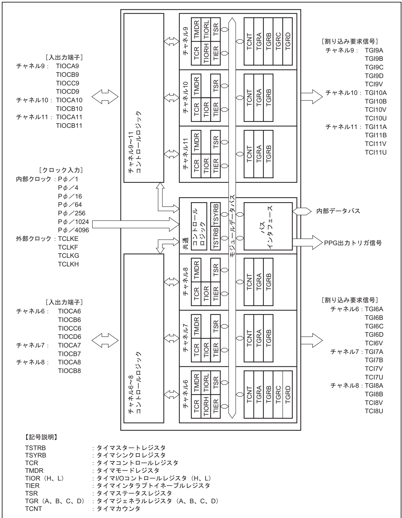
図 13.2 TPU (ユニット1) のブロック図
