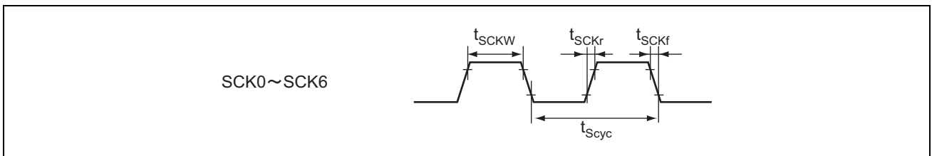
図 27.33 SCK クロック入力タイミング
