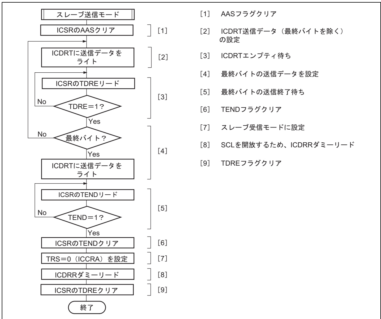
図 18.16 スレーブ送信モードフローチャート例
