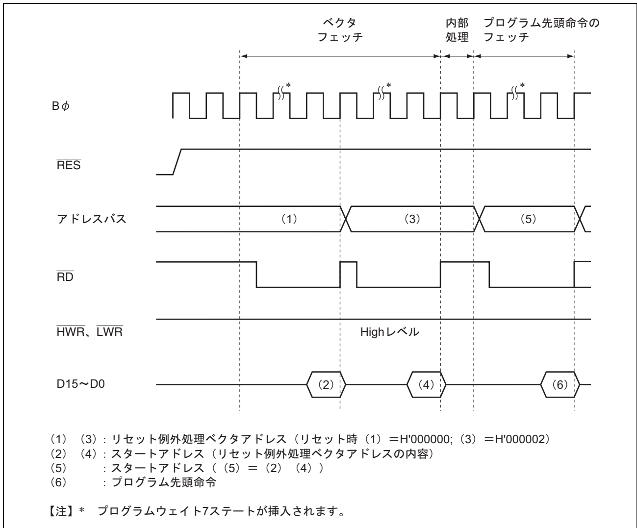
図 6.2 リセットシーケンス (アドバンストモード/内蔵 ROM 無効/外部 16 ビットアクセス空間)
