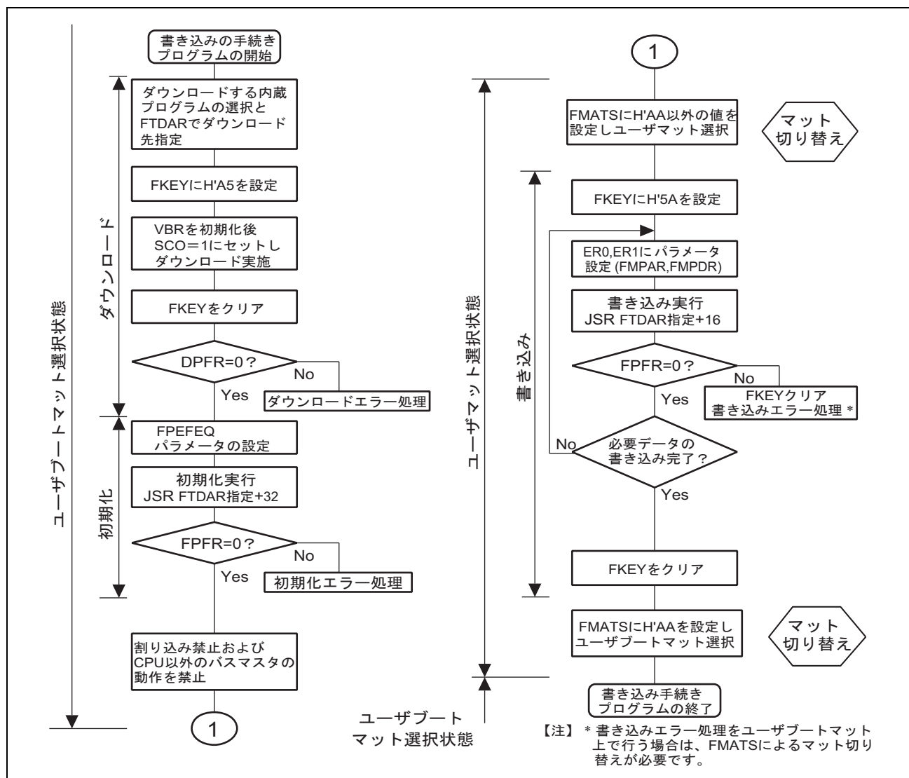
図 22.14 ユーザーブートモードでのユーザーマットへの書き込み手順
