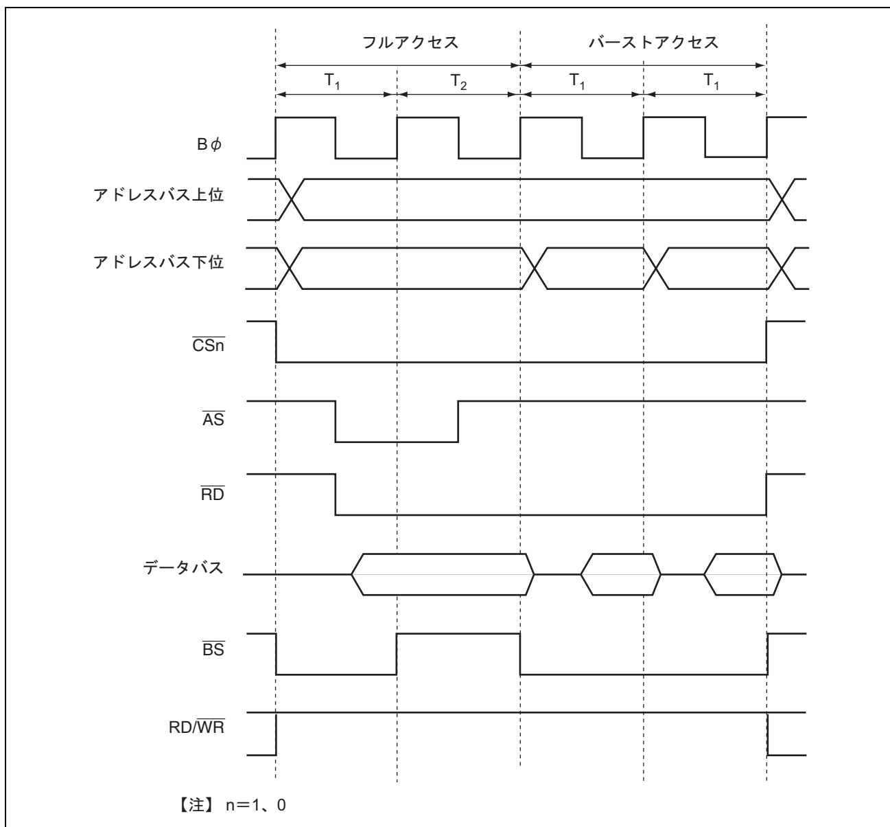
図 9.29 バースト ROM アクセスタイミング例 (ASTn=0、バーストサイクル1ステート)
