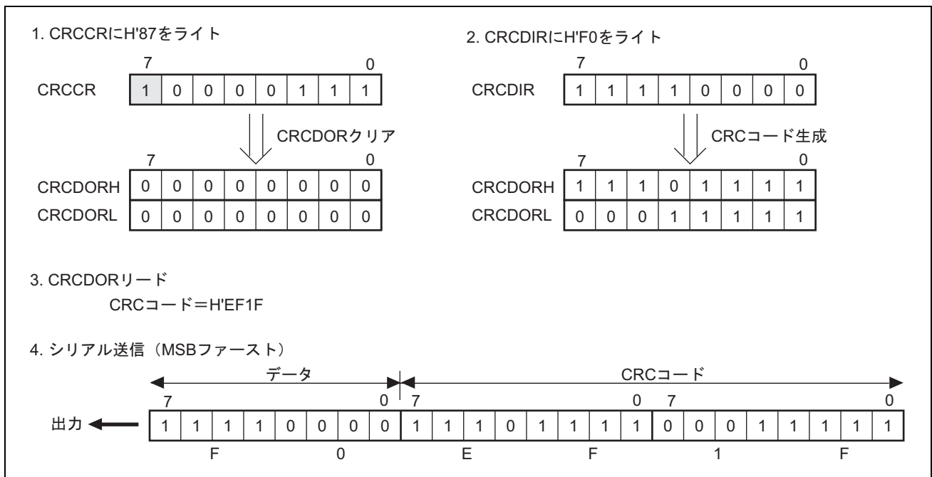
図 17.45 MSB ファーストでのデータ送信
