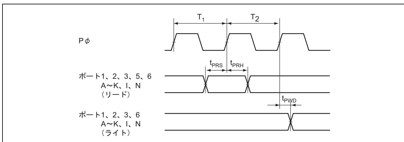
図 27.25 I/O ポート入出力タイミング
