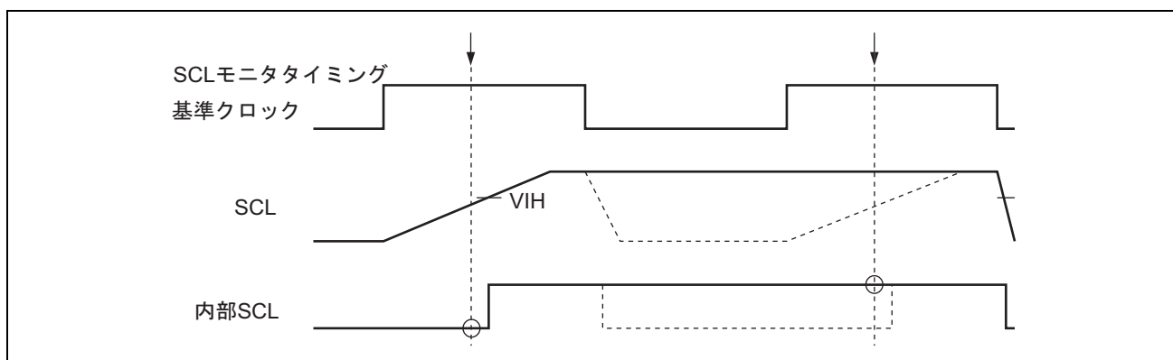
図 18.18 ビット同期回路のタイミング
