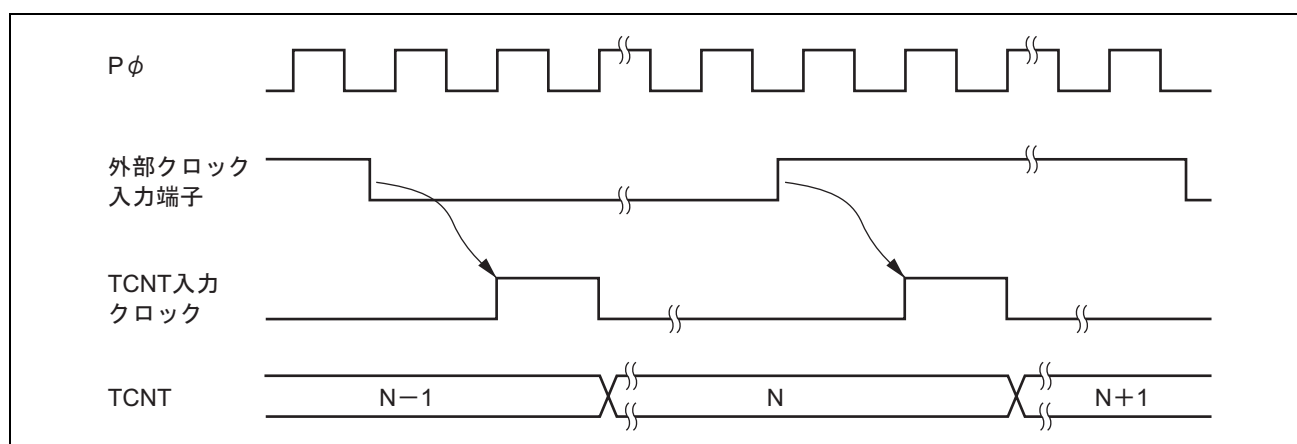
図 15.8 外部クロック動作時のカウントタイミング
