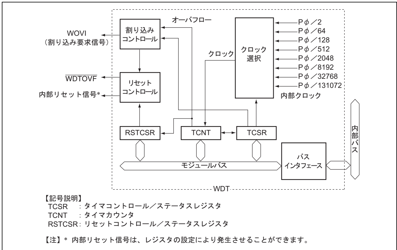
図 16.1 WDT のブロック図
