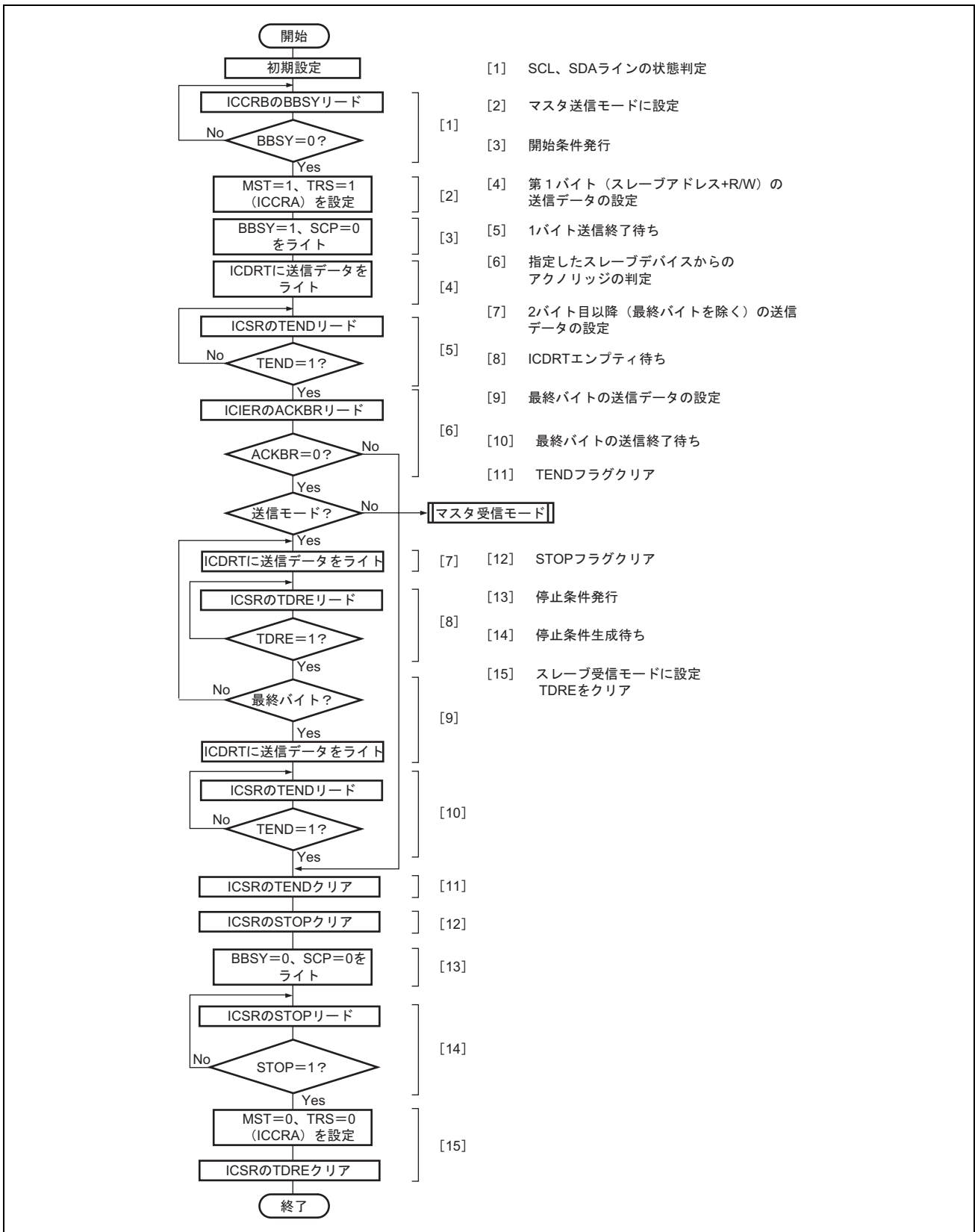
図 18.14 マスタ送信モードのフローチャート例
