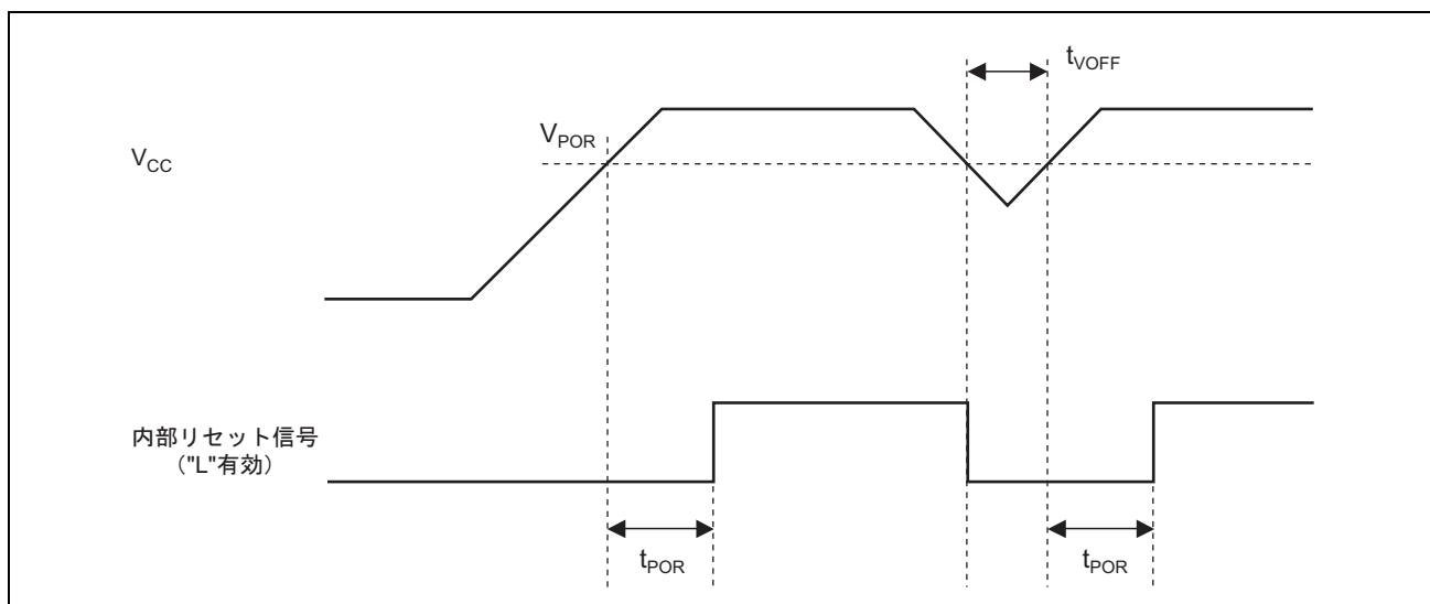
図 27.40 パワーオンリセットタイミング
