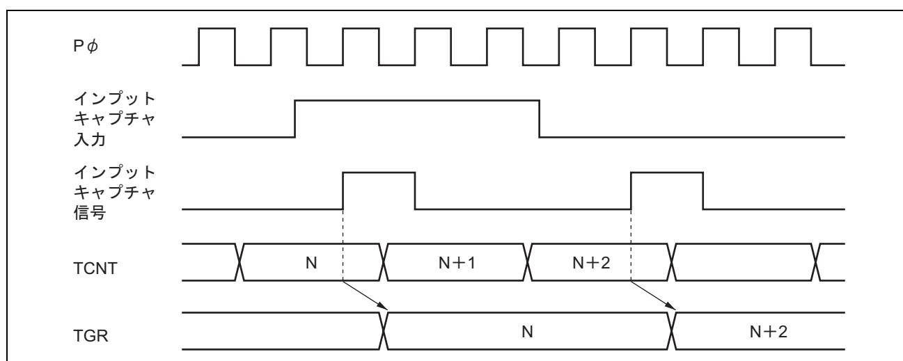
図 13.34 インプットキャプチャ入力信号タイミング
