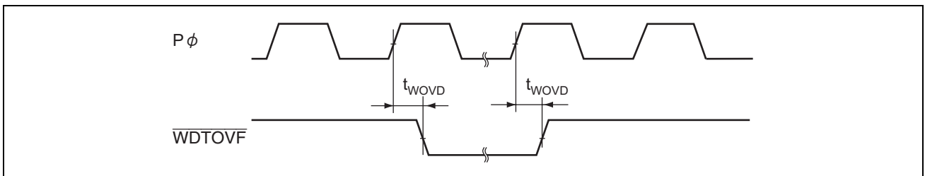
図 27.32 WDT 出カタイミング
