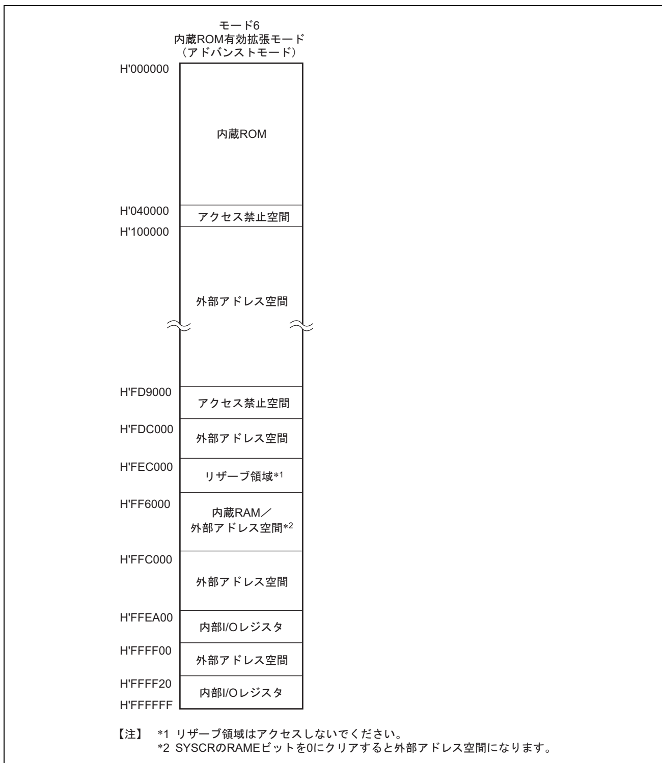
図 3.3 H8SX/1641、H8SX/1641L の各動作モードのアドレスマップ (2)
