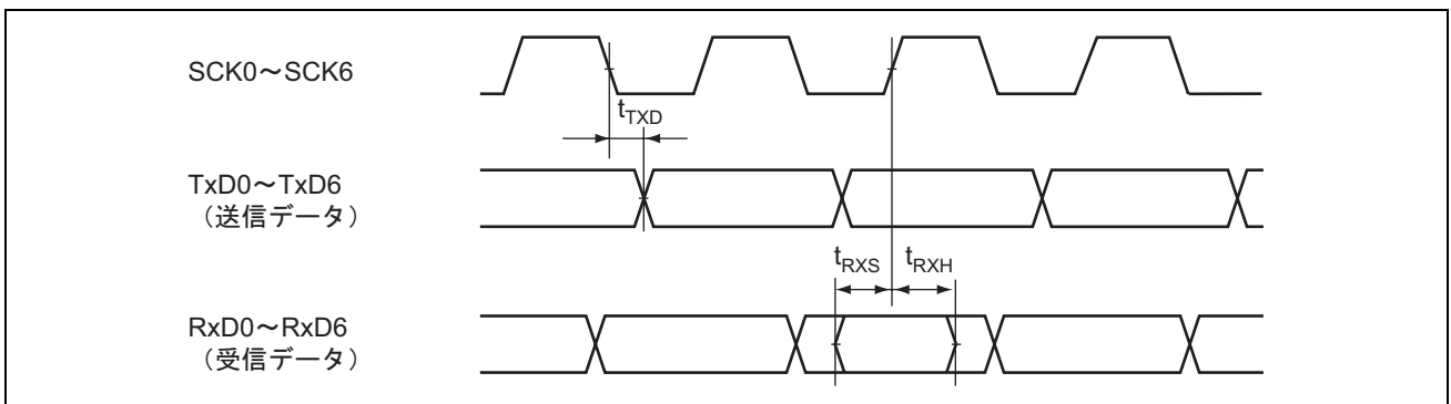
図 27.34 SCI 入出カタイミング/クロック同期式モード
