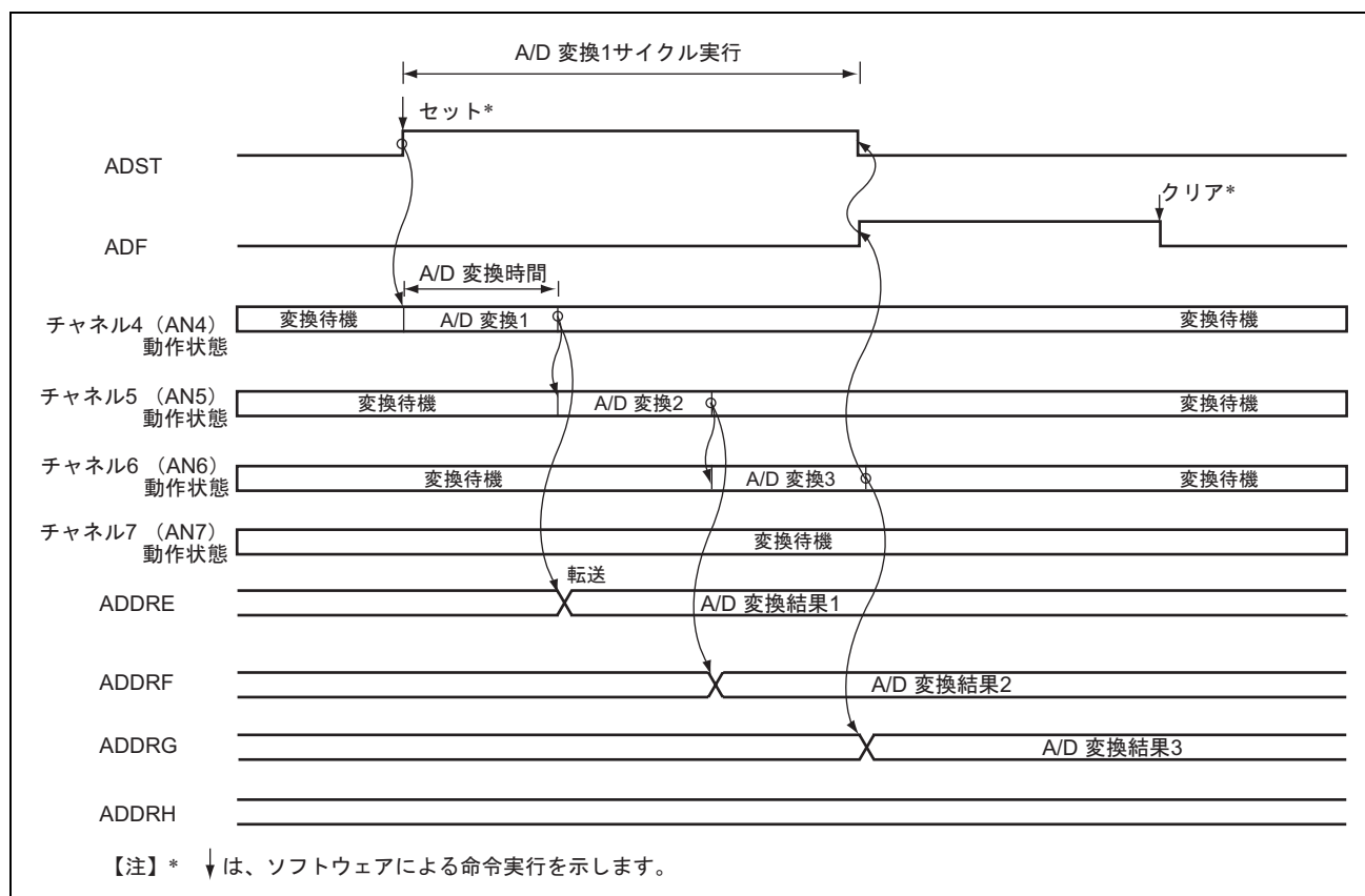
図 19.6 A/D 変換器の動作例（1サイクルスキャンモード、AN4～AN6の3チャンネル選択時）
