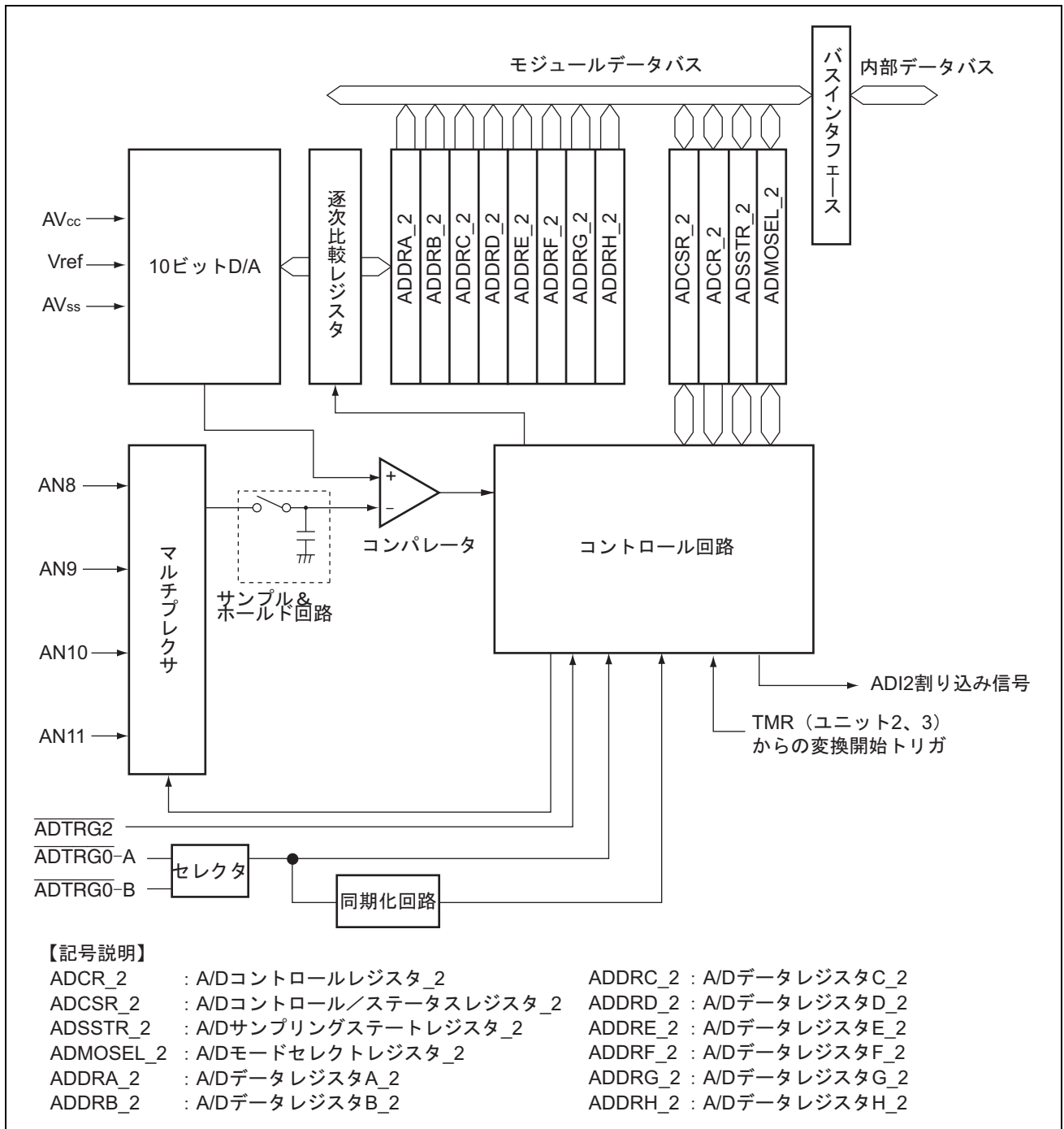
図 19.3 A/D 変換器 (ユニット 2/AD_2) のブロック図
