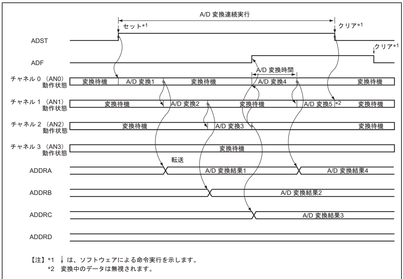
図 19.5 A/D 変換器の動作例（連続スキャンモード、AN0～AN2 の 3 チャンネル選択時）
