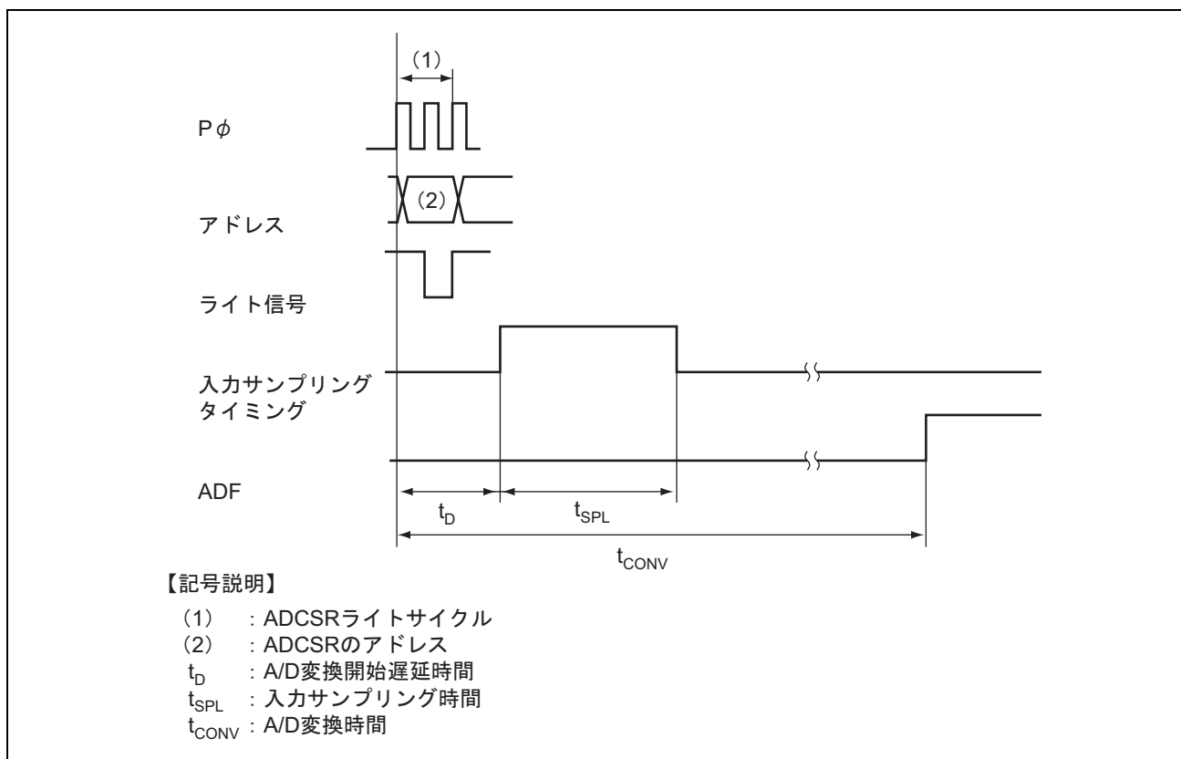
図 19.7 A/D 変換タイミング
