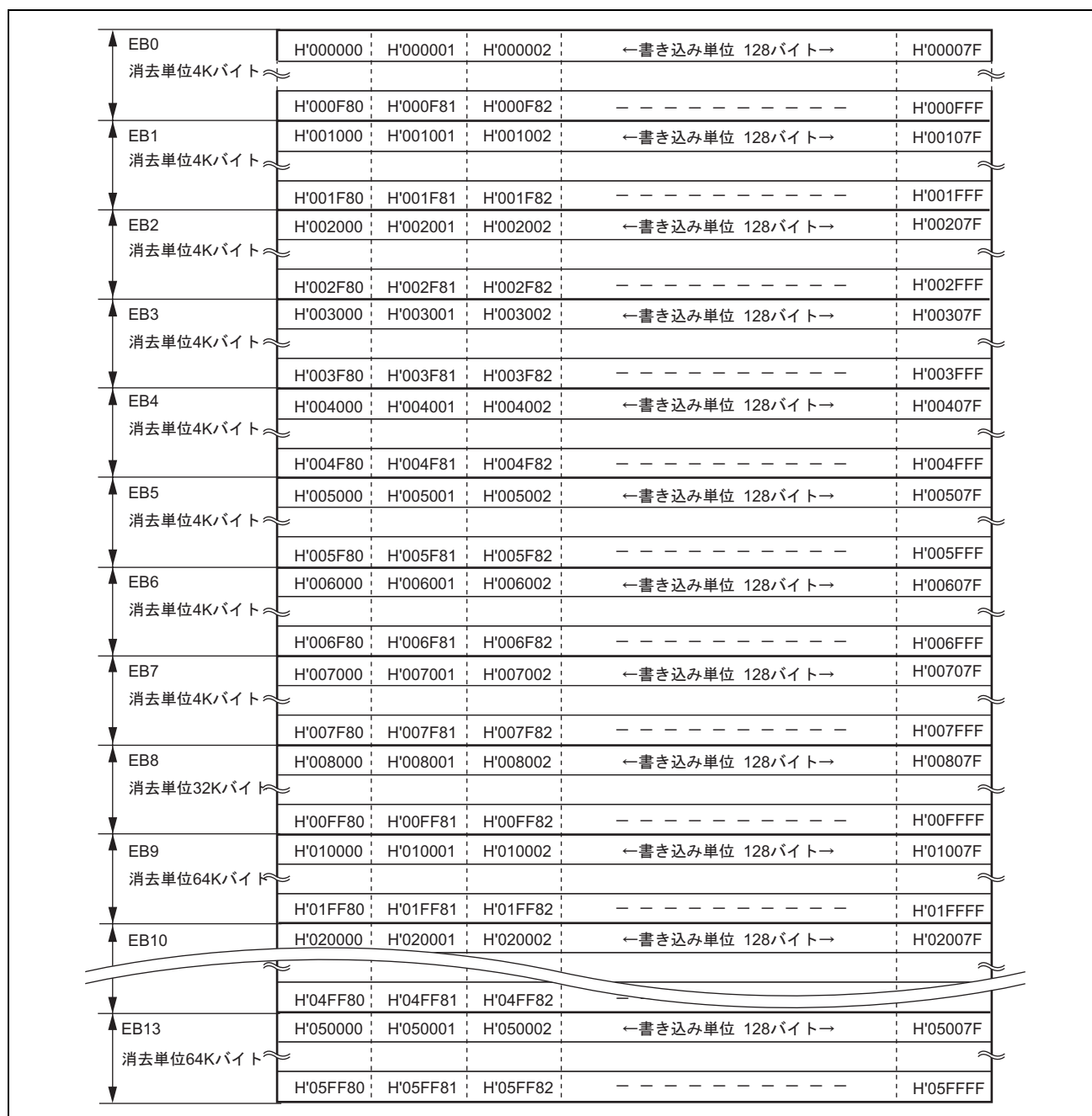
図 22.4 (2) H8SX/1643 のユーザマットのブロック構成
