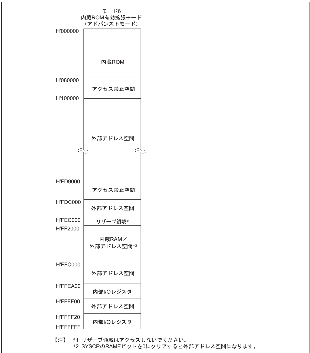
図 3.1 H8SX/1645、H8SX/1645L の各動作モードのアドレスマップ (2)
