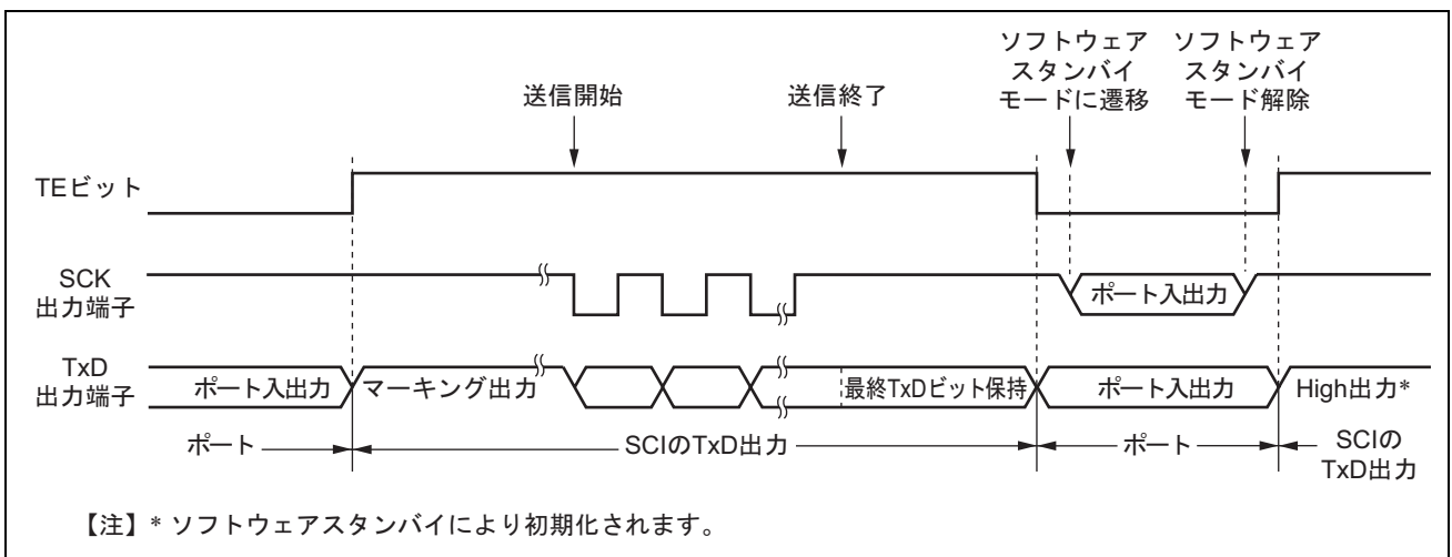
図 17.41 ソフトウェアスタンバイモード遷移時のポートの端子状態 (内部クロック、クロック同期送信)
