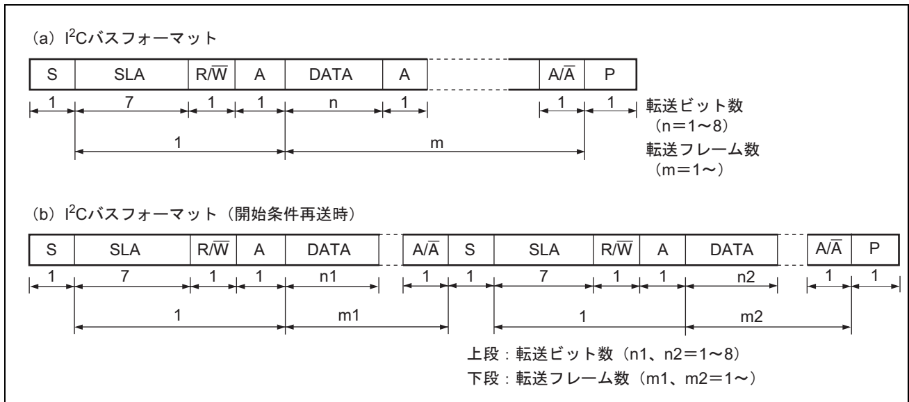
図 18.3 I 2 C バスフォーマット
