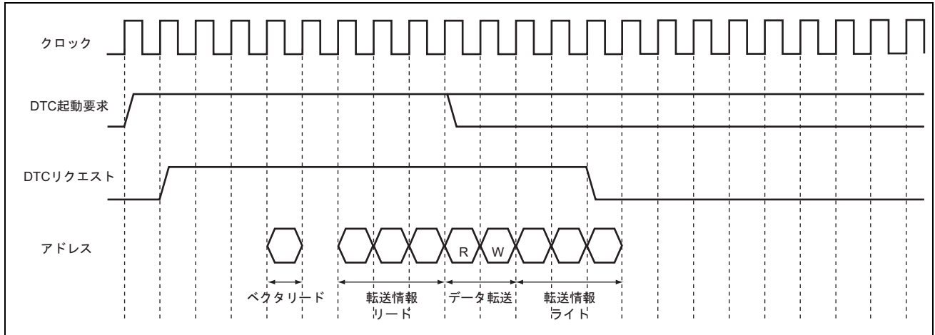
図 11.11 DTC の動作タイミング例 (ショートアドレスモード、ノーマル転送モード、リピート転送モード)
