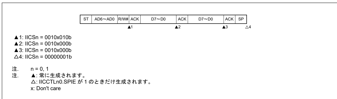
図 22.37 スレーブデバイスの拡張コード受信動作 (IICCTLn0.WTIM が 0 の場合)
