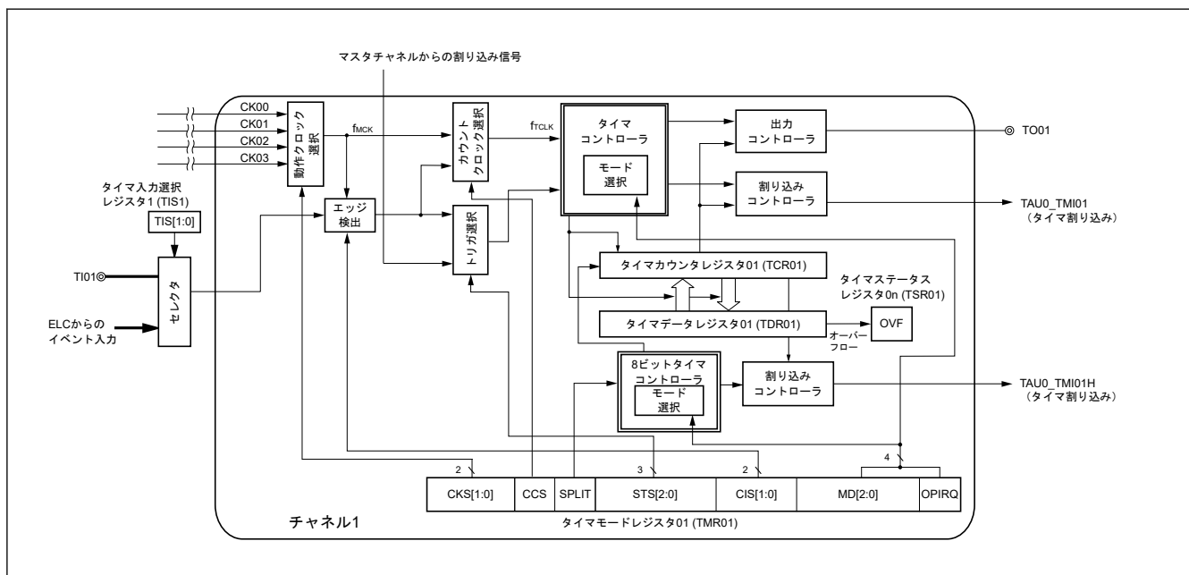
図 17.14 タイマアレユニット 0 のチャンネル 1 の内部ブロック図
