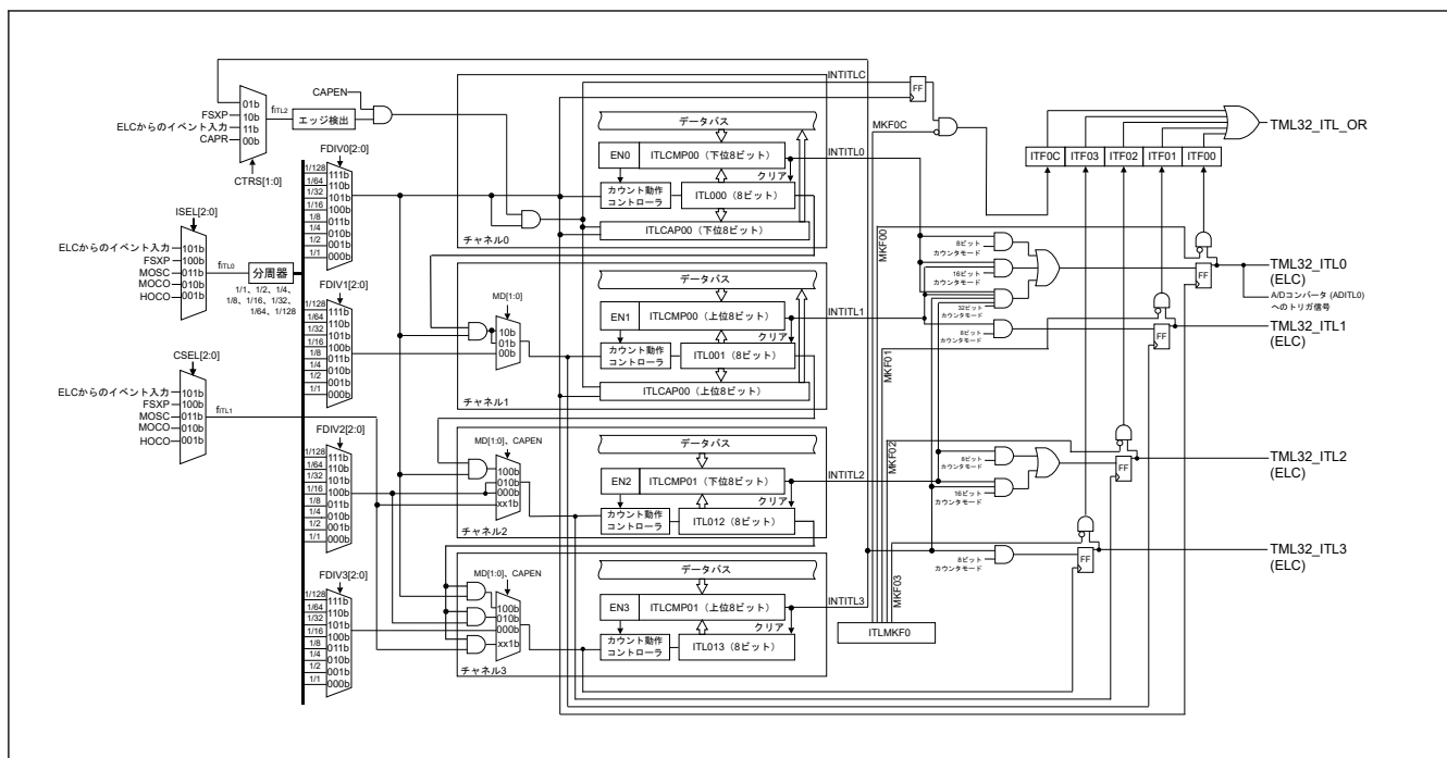
図 18.5 32 ビットインターバルタイマのブロック図
