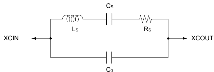
図 8.7 32.768 kHz 水晶振動子の等価回路
