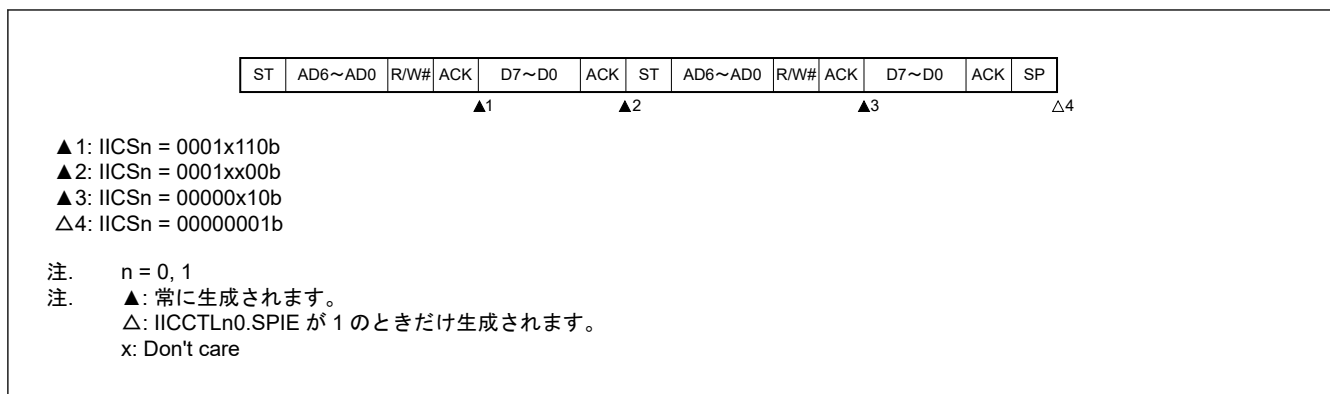
図 22.36 通常アクセスの後のスレーブデバイスの動作、一致しない (IICCTLn0.WTIM = 1)
