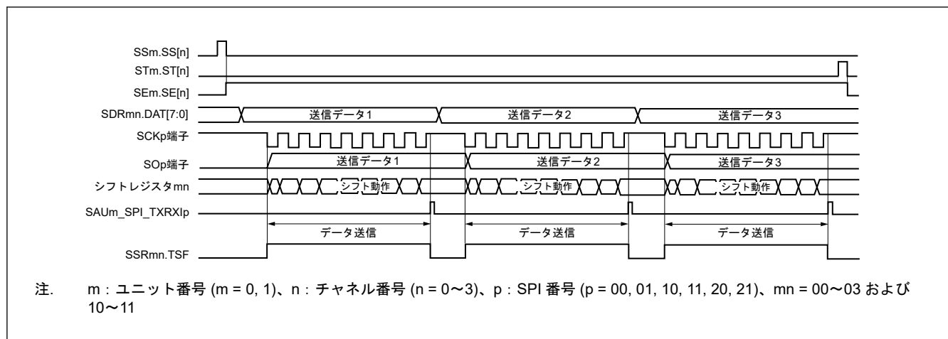
図 21.17 スレーブ送信のタイミング（シングル送信モードの場合）（タイプ1 : SCRmn.DCP[1:0] = 00b）
