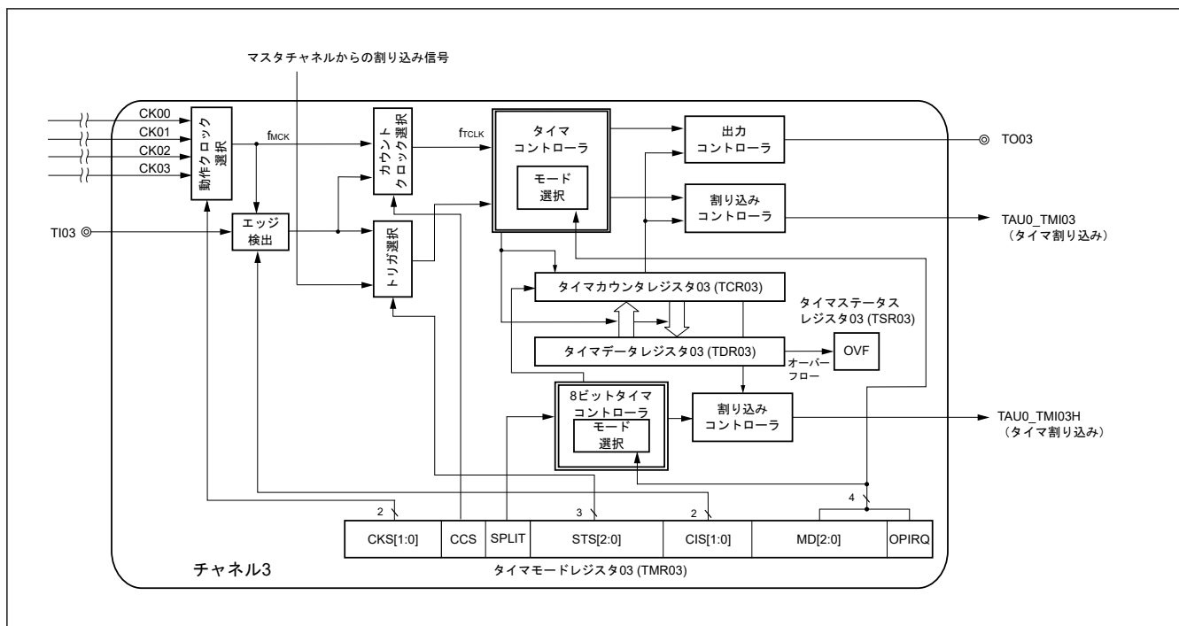
図 17.16 タイマアレiyユニット 0 のチャンネル 3 の内部ブロック図
