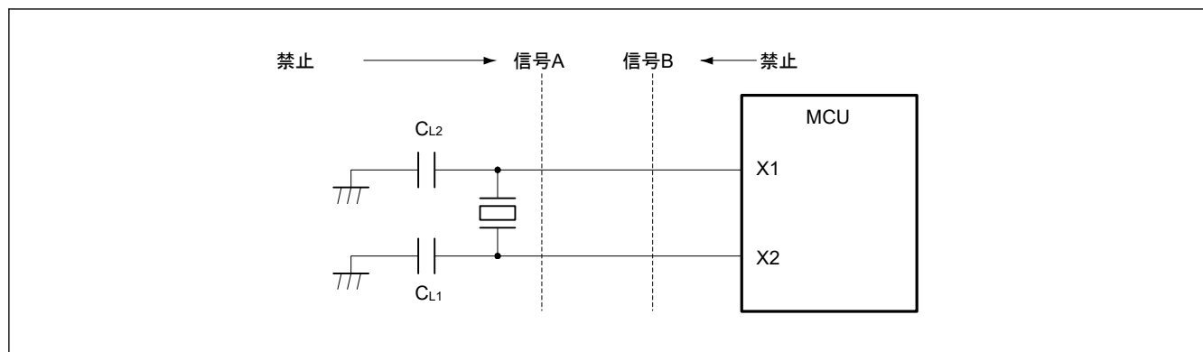
図 8.10 発振回路部のボード設計に関する信号のルーティング
