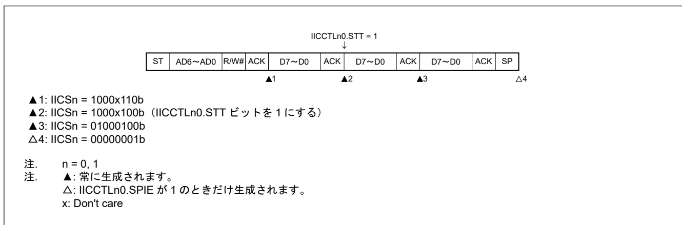
図 22.58 リスタートコンディションの生成を試みた時に Low レベルデータによりアービトレーションロストが発生した場合の動作 (IICCTLn0.WTIM = 1)
