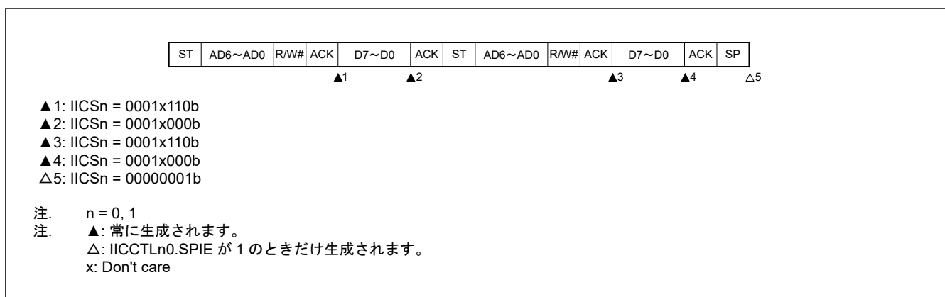
図 22.31 通常アクセスの後のスレーブデバイスの動作、SVAn と一致する (IICCTLn0.WTIM = 0)
