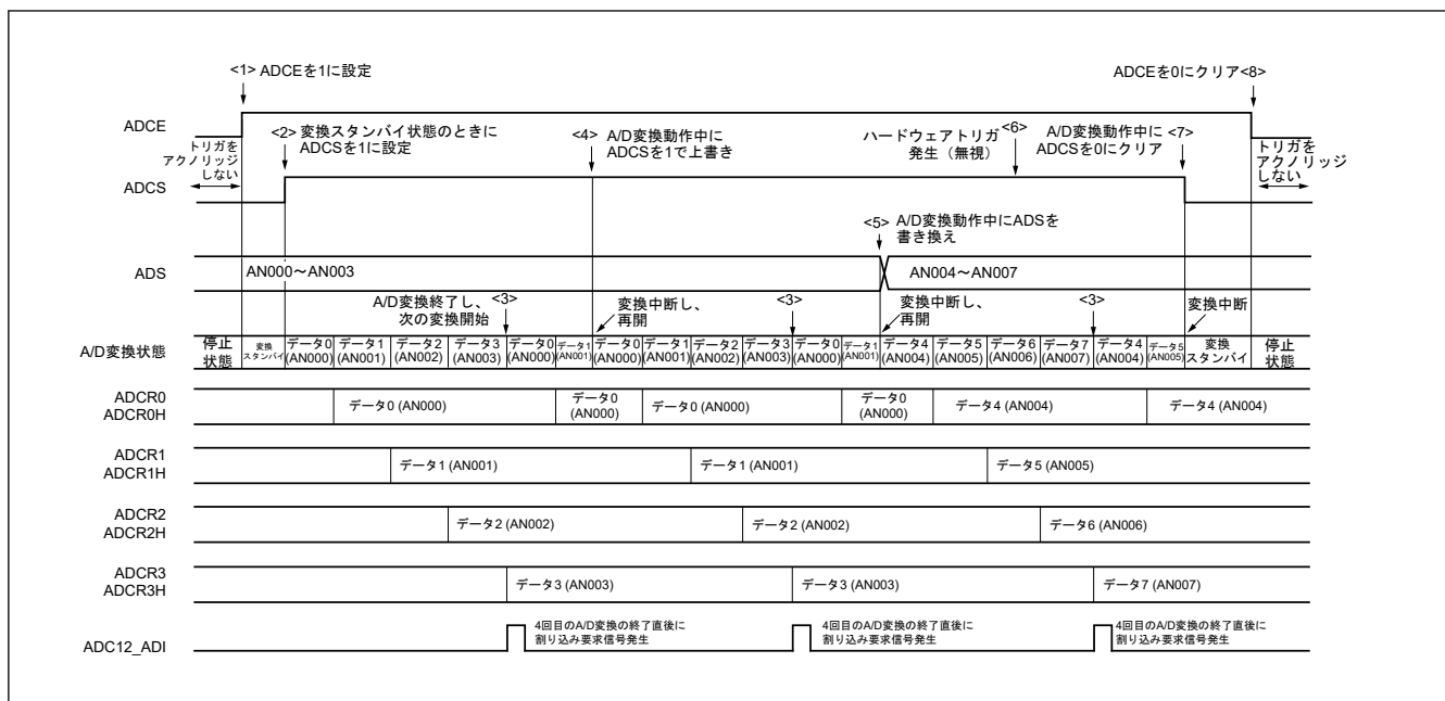
図 25.10 ソフトウェアトリガ待機なしモード（スキャンモード、連続変換モード）動作タイミングの例
