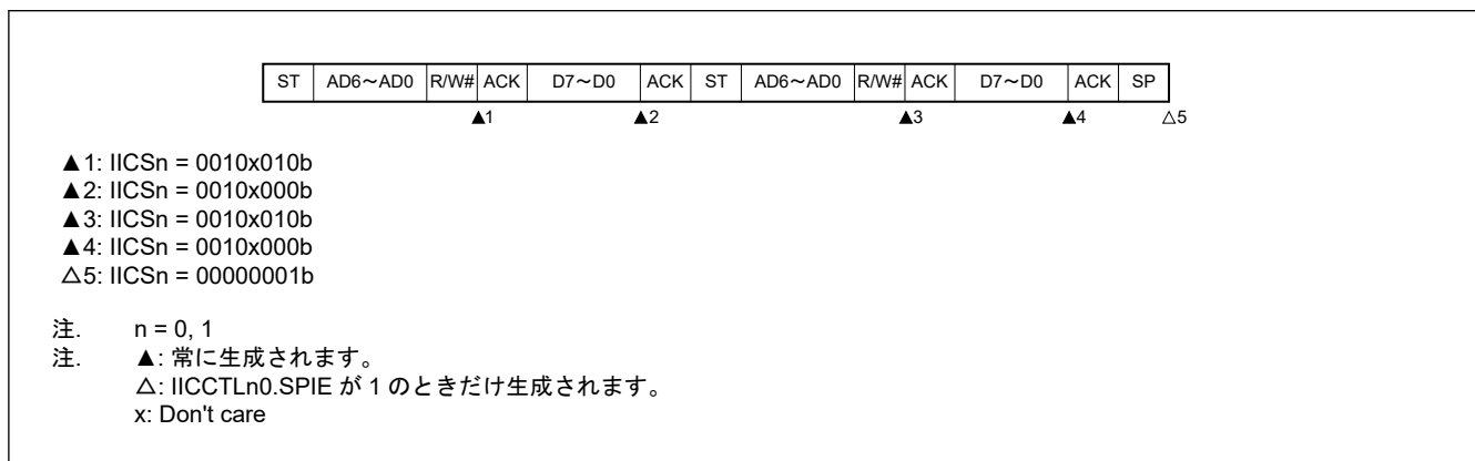
図 22.41 コードアクセスの後のスレーブデバイスの動作、拡張コードと一致する (IICCTLn0.WTIM = 0)
