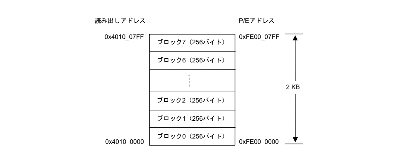
図 28.3 データフラッシュメモリマッピング
