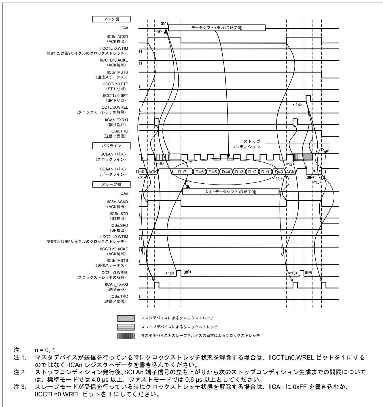
図 22.65 マスタデバイスとスレーブデバイス間通信の例（マスタデバイスとスレーブデバイスが第 9 サイクルでクロックストレッチを挿入する場合。）(3/4)
