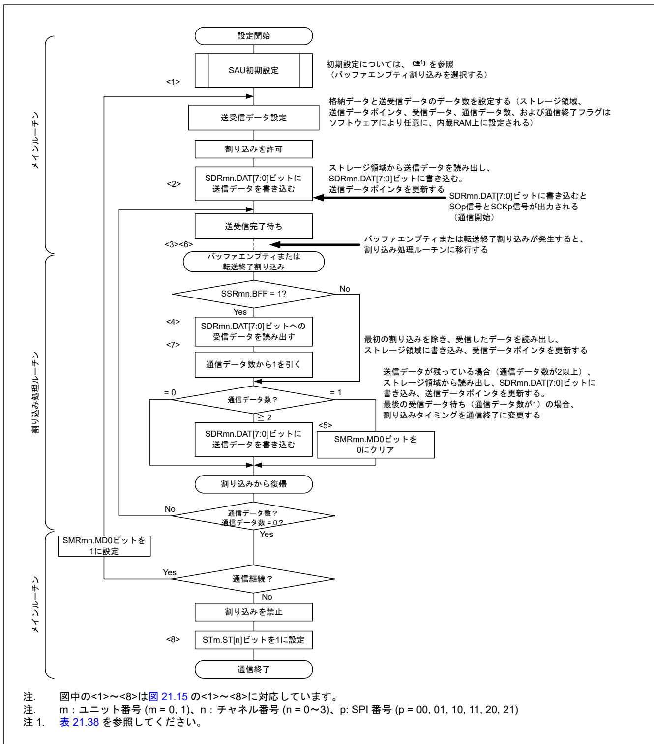
図 21.16 マスタ送受信のフローチャート (連続送受信モード時)
