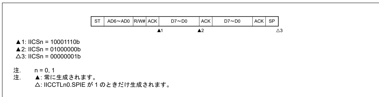
図 22.52 データ転送時にアービトレーションロストが発生した場合の動作（IICCTLn0.WTIM が 0 の場合）
