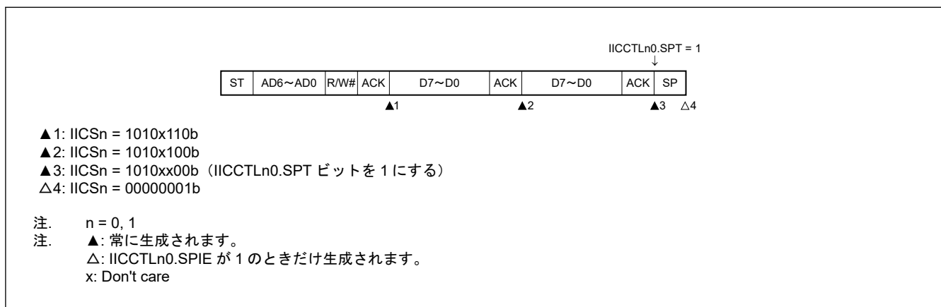
図 22.28 マスタデバイスの拡張コード送信動作 (IICCTLn0.WTIM が 1 の場合)
