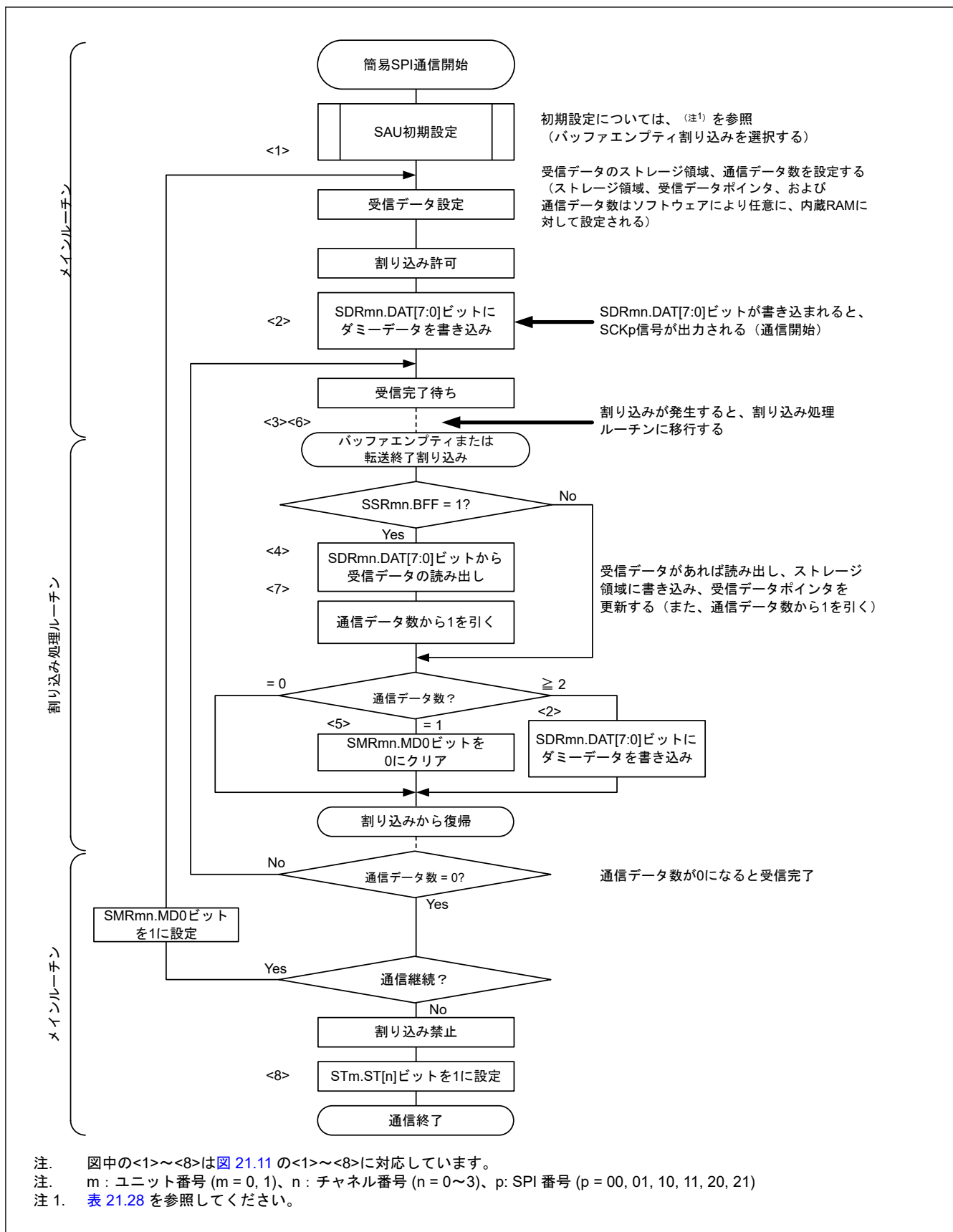
図 21.12 マスタ受信のフローチャート (連続受信モード時)
