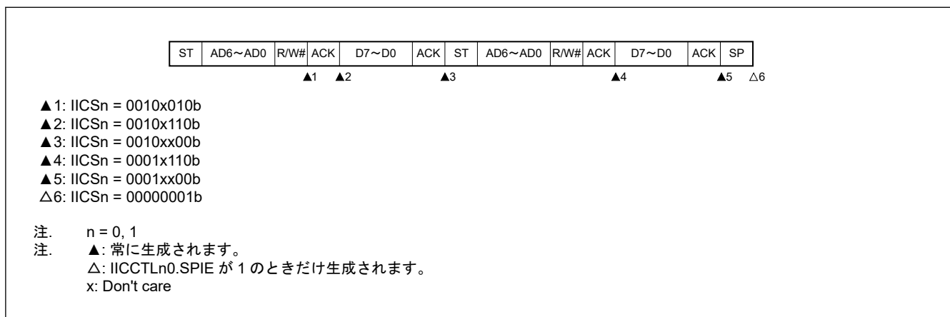
図 22.40 コードアクセスの後のスレーブデバイスの動作、SVAn と一致する (IICCTLn0.WTIM = 1)
