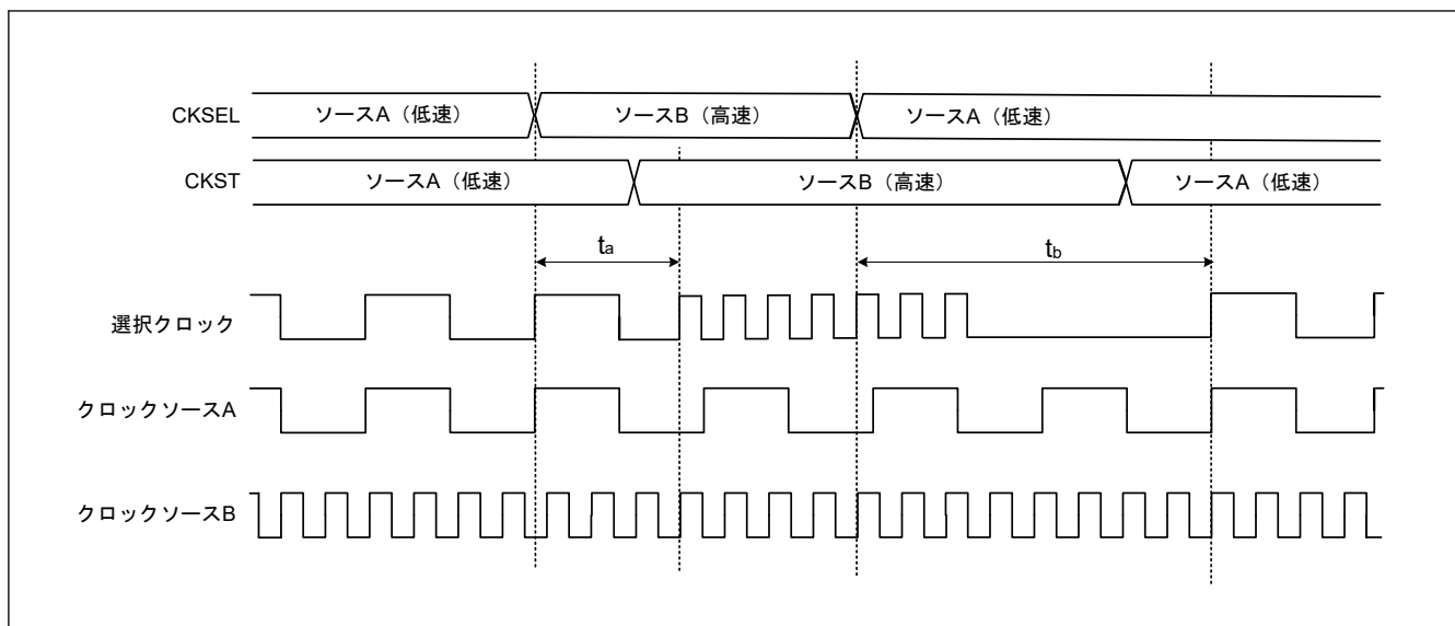
図 8.9 クロックソース切り替えのタイミング
