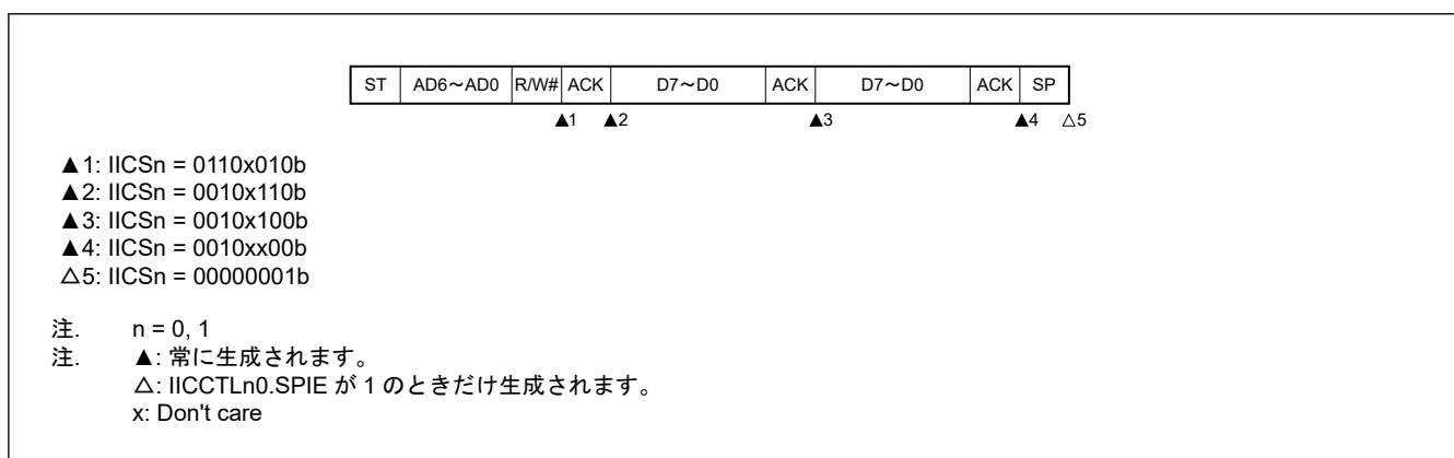
図 22.49 拡張コード送信時のアービトレーションロスト（IICCTLn0.WTIM が 1 の場合）
