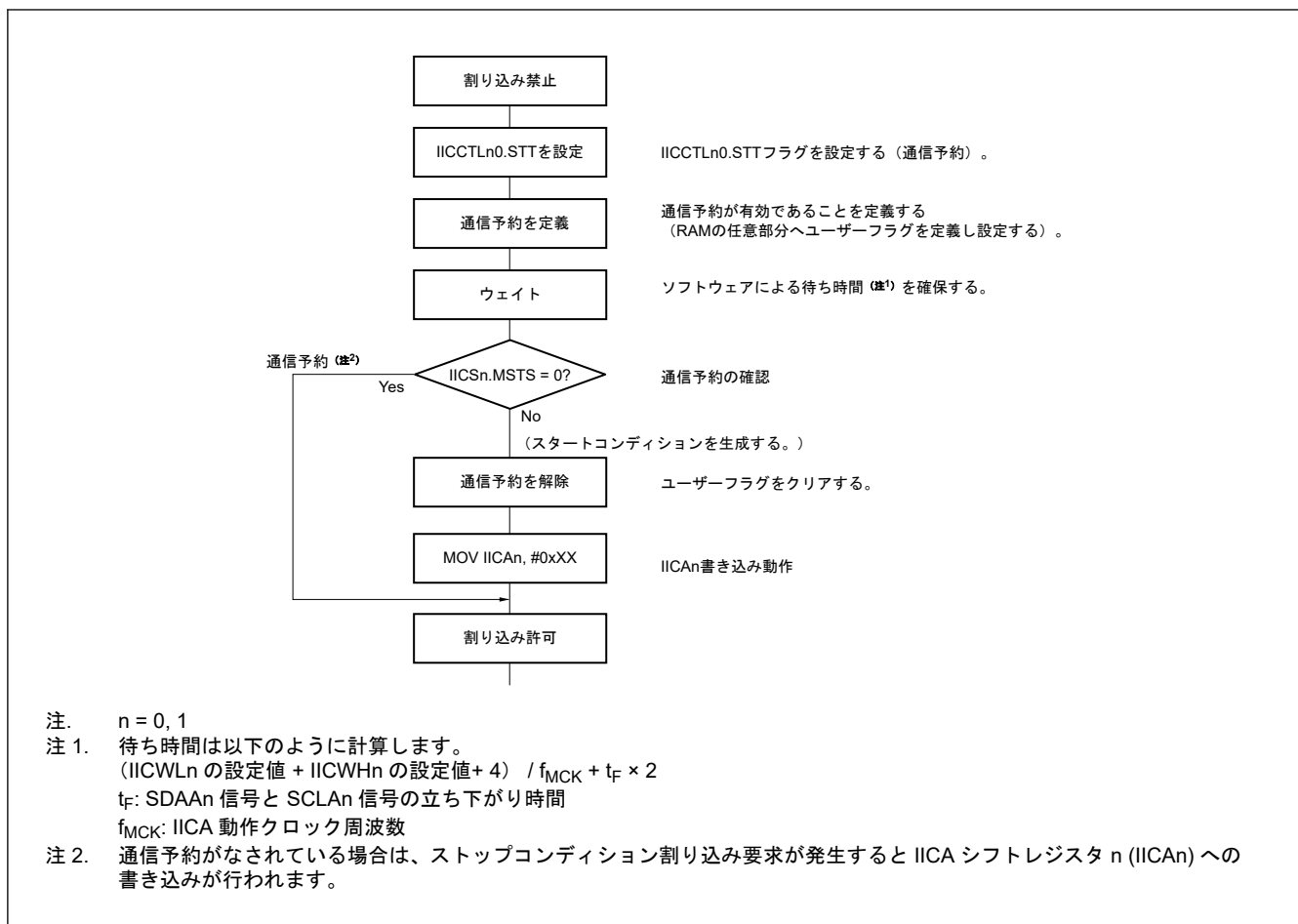
図 22.15 通信予約の処理手順
