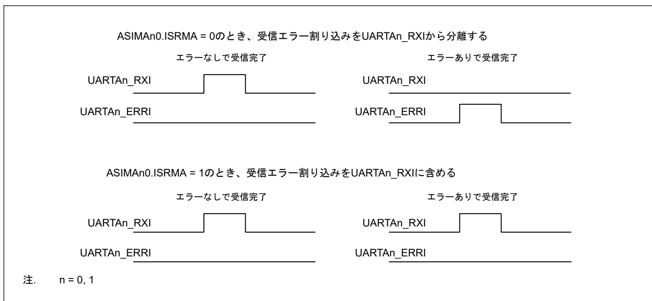
図 23.8 ASIMAn0.ISRMA 設定値によって変化する割り込み出力
