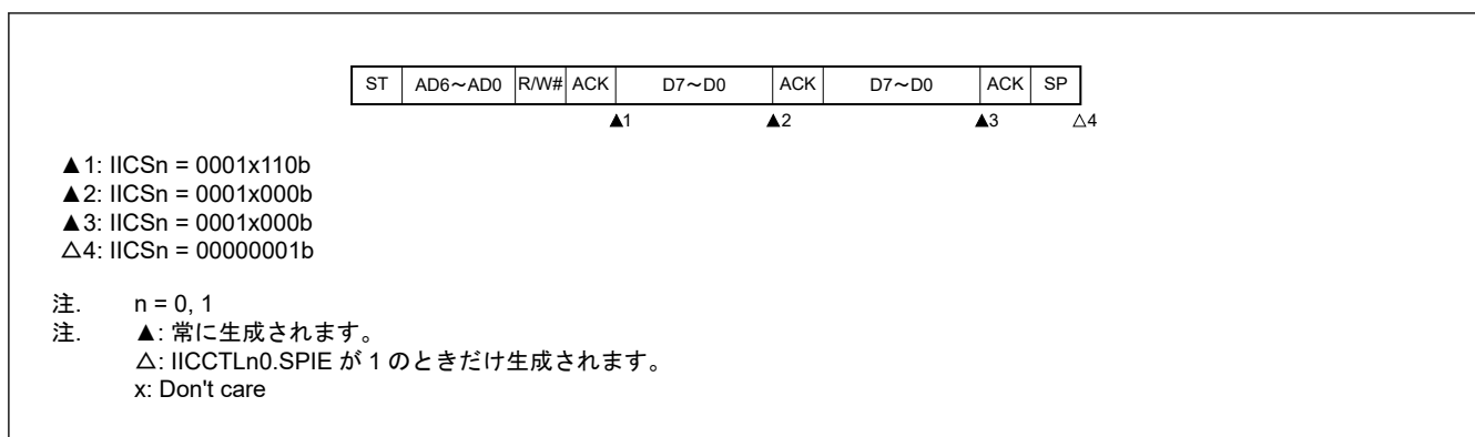
図 22.29 スレーブデバイスのスレーブアドレスデータ受信動作 (IICCTLn0.WTIM が 0 の場合)
