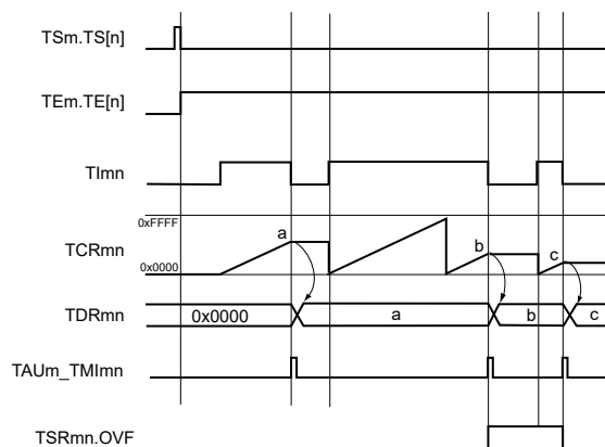
図 17.46 入力信号の High/Low レベル幅を測定する動作の基本タイミング例
