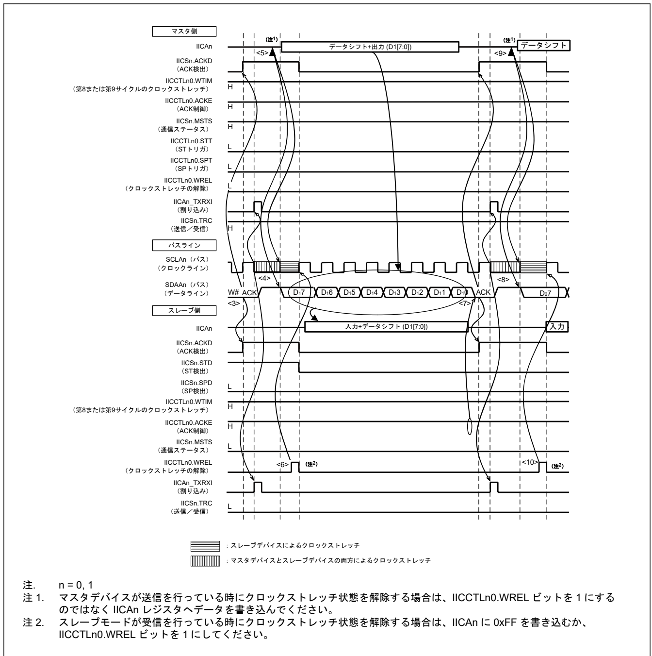
図 22.64 マスタデバイスとスレーブデバイス間通信の例 (マスタデバイスとスレーブデバイスが第 9 サイクルでクロックストレッチを挿入する場合。) (2/4)
