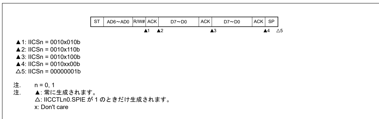
図 22.38 スレーブデバイスの拡張コード受信動作 (IICCTLn0.WTIM が 1 の場合)
