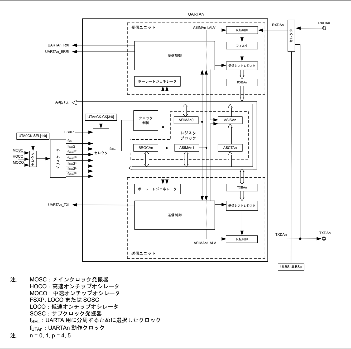
図 23.1 UARTAn のブロック図
