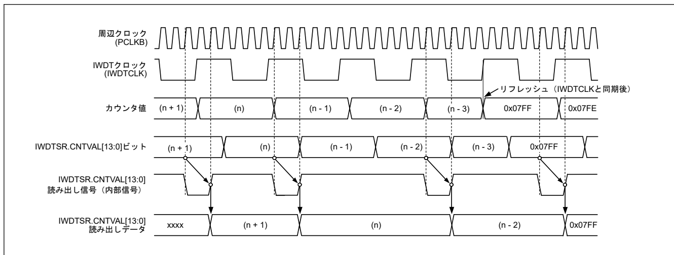
図 20.5 IWDTC ダウンカウンタ値の読み出し処理 ( OFS0.IWDTCCKS[3:0] = 0000b 、 OFS0.IWDTCCTOPS[1:0] = 11b の場合)
