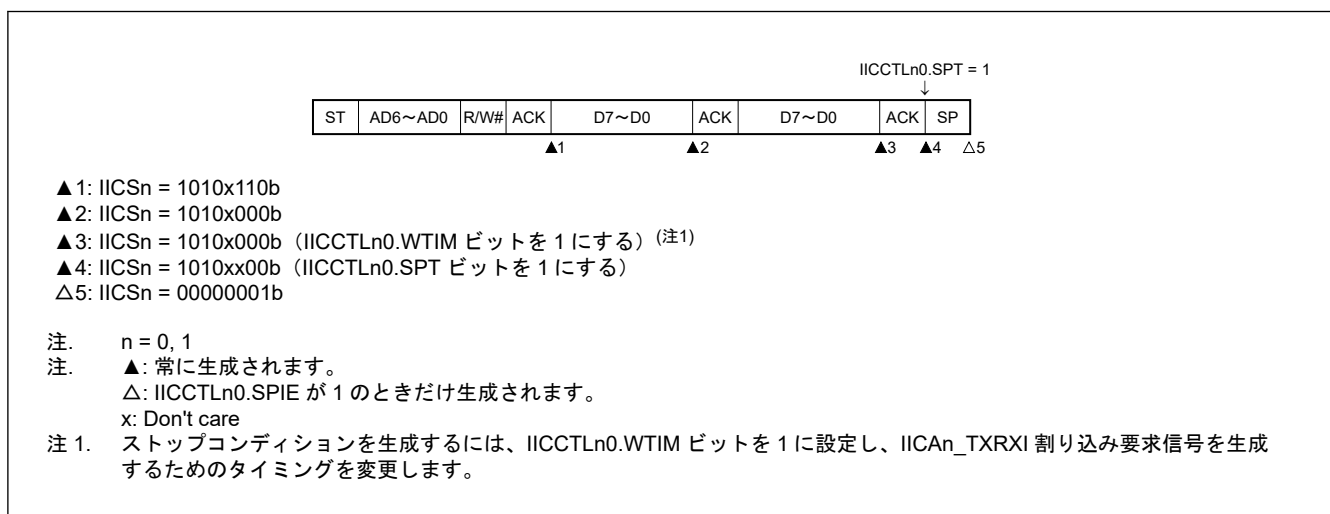
図 22.27 マスタデバイスの拡張コード送信動作 (IICCTLn0.WTIM が 0 の場合)
