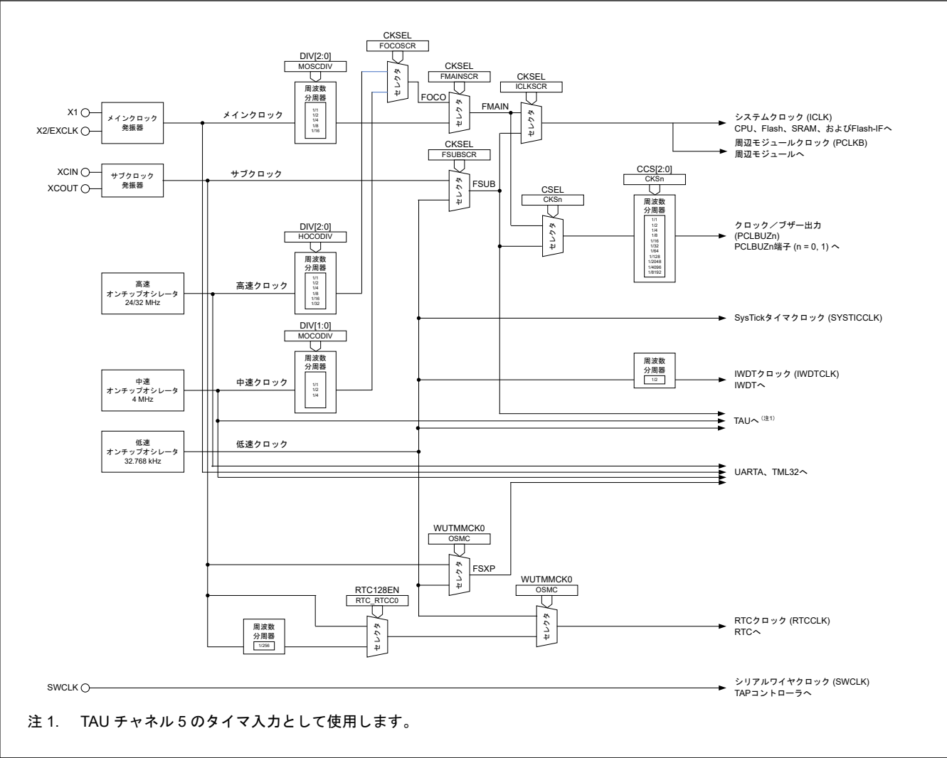
図 8.1 クロック発生回路のブロック図 (64、48、32 ピン)
