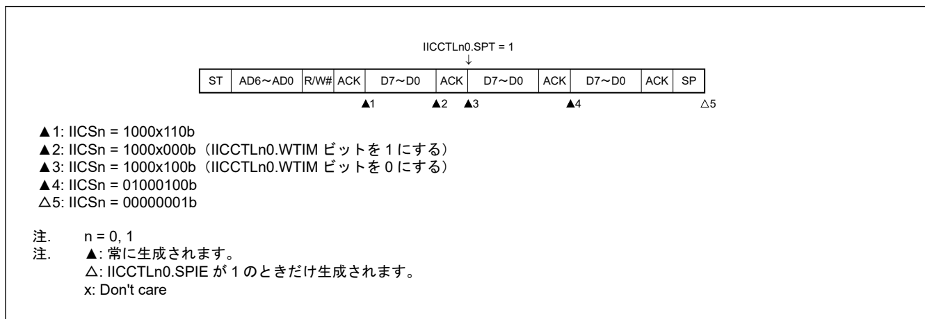
図 22.61 ストップコンディションを生成しようとしたときの S の Low レベルデータのためにアービトレーションロストが発生した場合の動作 (IICCTLn0.WTIM = 0)
