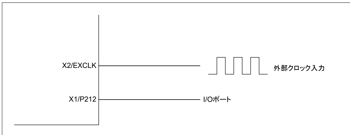
図 8.5 外部クロックの等価回路
