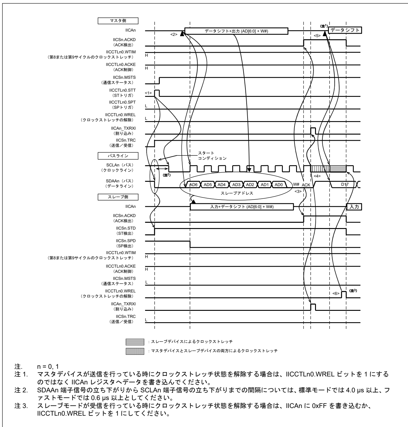
図 22.63 マスタデバイスとスレーブデバイス間通信の例（マスタデバイスとスレーブデバイスが第9サイクルでクロックストレッチを挿入する場合。）(1/4)
