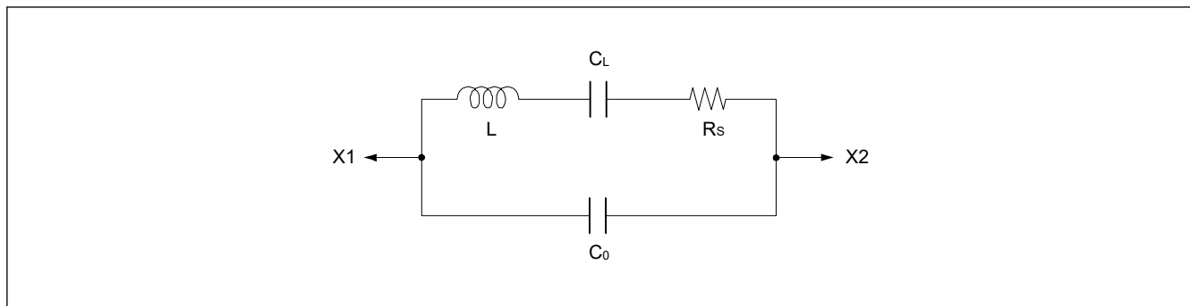
図 8.4 発振子の等価回路
