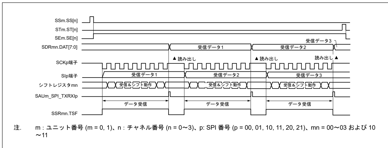
図 21.21 スレーブ受信のタイミング (シングル受信モードの場合) (タイプ 1 : SCRmn.DCP[1:0] = 00b)
