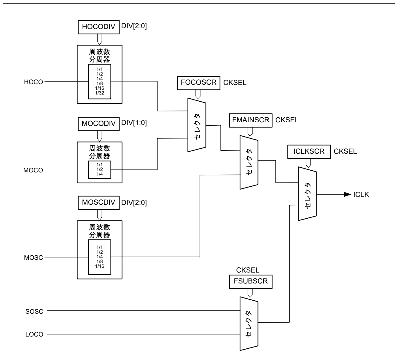
図 8.8 クロックソースセレクタのブロック図
