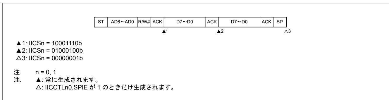
図 22.53 データ転送時にアービトレーションロストが発生した場合の動作（IICCTLn0.WTIM が 1 の場合）
