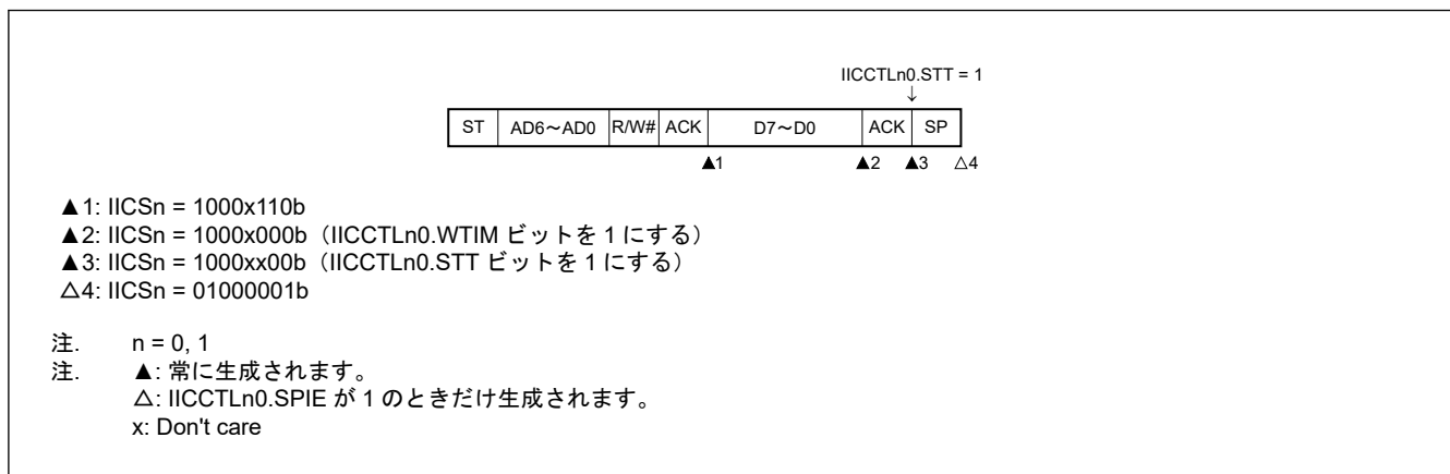
図 22.59 リスタートコンディションの生成を試みた時にストップコンディションによりアービトレーションロストが発生した場合の動作 (IICCTLn0.WTIM = 0)
