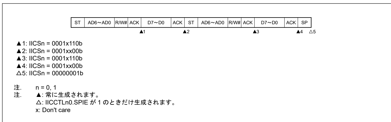
図 22.32 通常アクセスの後のスレーブデバイスの動作、SVAn と一致する (IICCTLn0.WTIM = 1)
