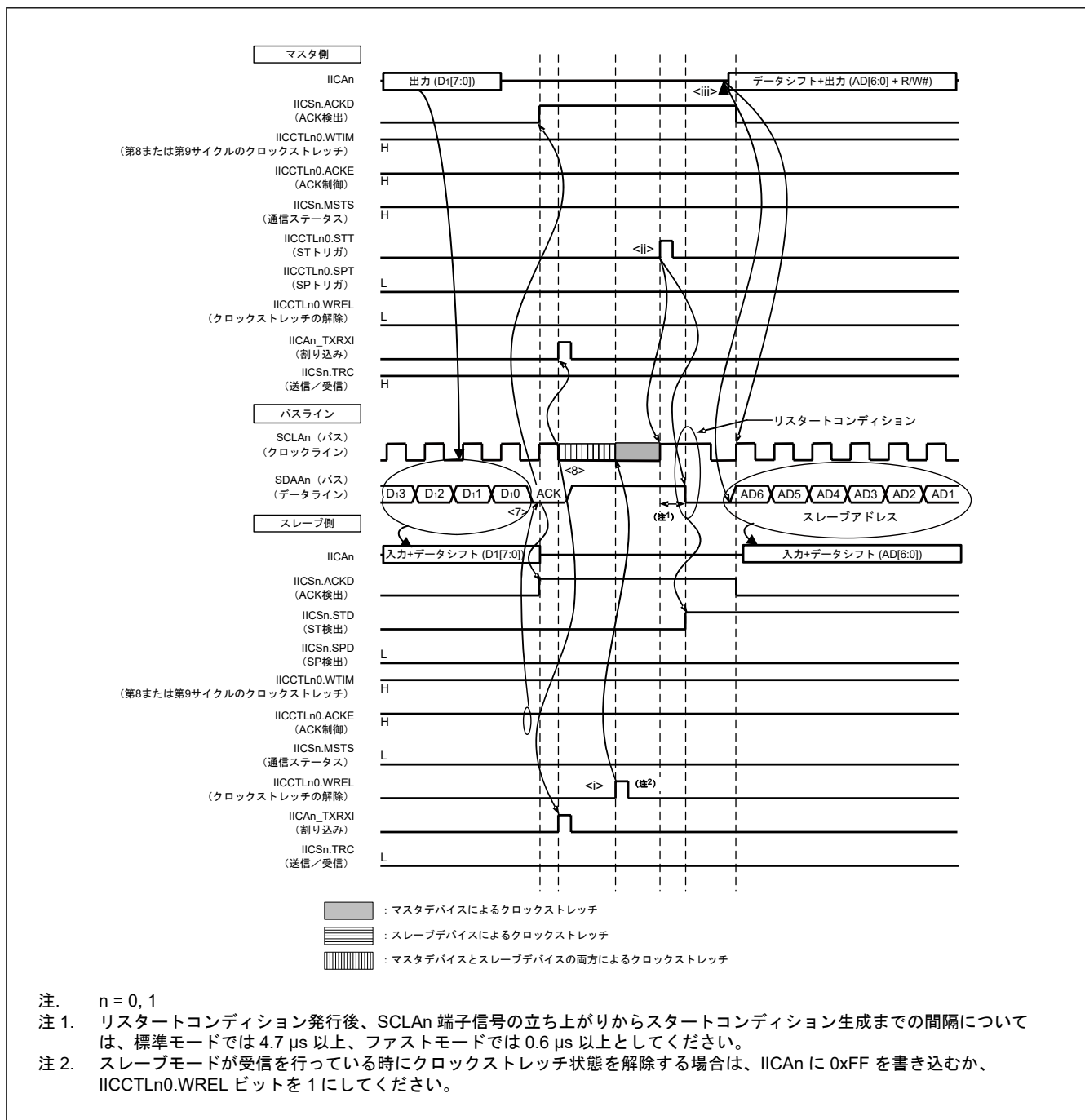
図 22.66 マスタデバイスとスレーブデバイス間通信の例（マスタデバイスとスレーブデバイスが第 9 サイクルでクロックストレッチを挿入する場合。） (4/4)
