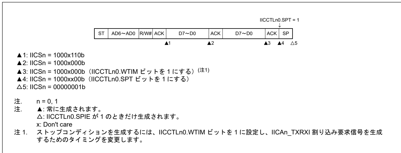
図 22.23 マスタデバイスの動作 (受信/送信) (IICCTLn0.WTIM が 0 の場合)
