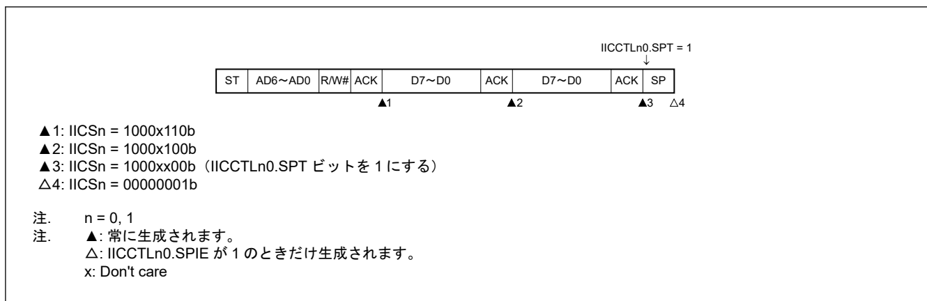
図 22.24 マスタデバイスの動作 (受信/送信) (IICCTLn0.WTIM が 1 の場合)
