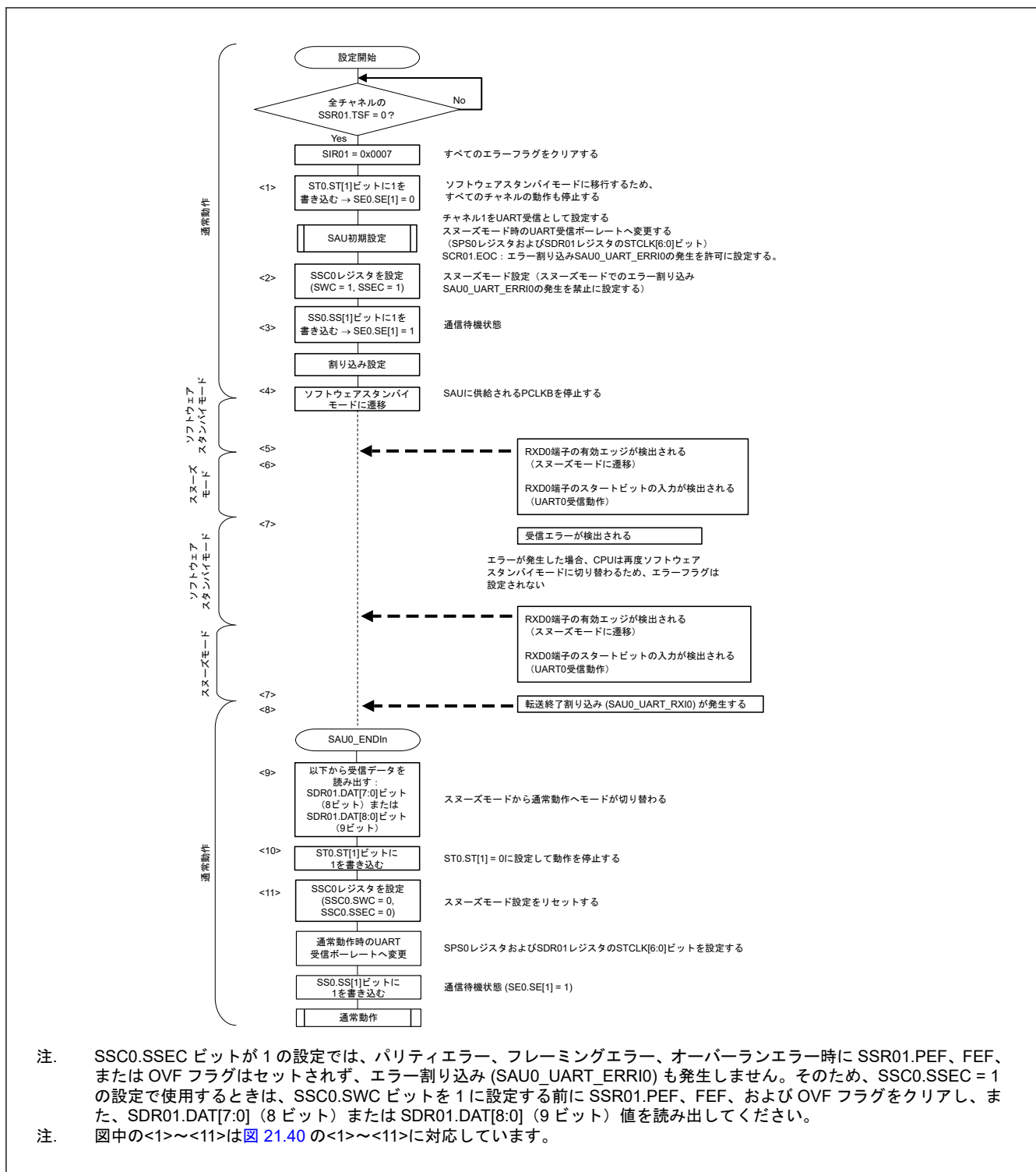
図 21.41 スレーブモード動作のフローチャート (SCR01.EOC = 1, SSC0.SSEC = 1)
