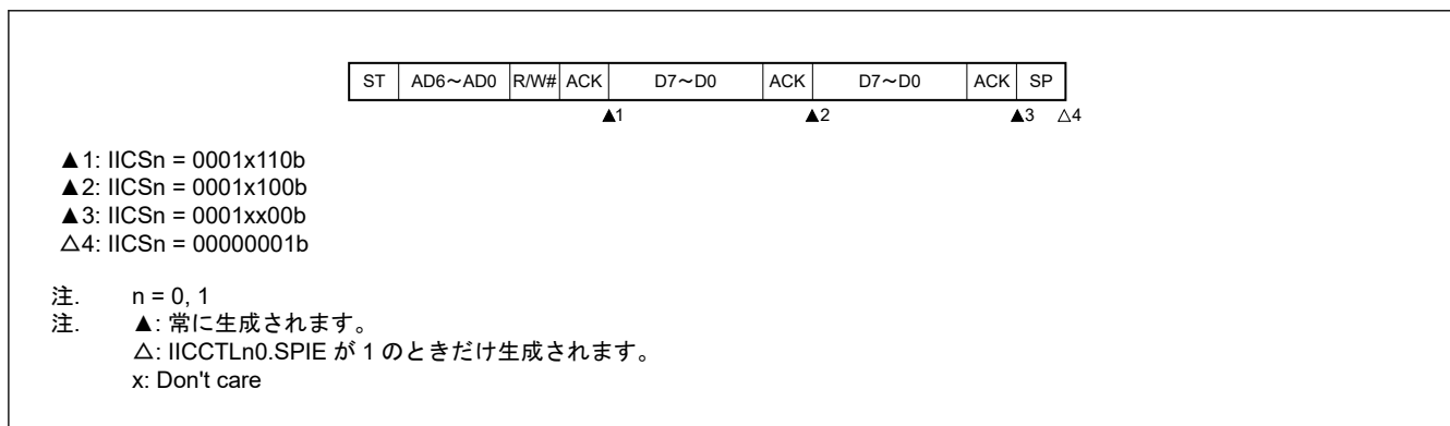
図 22.30 スレーブデバイスのスレーブアドレスデータ受信動作 (IICCTLn0.WTIM が 1 の場合)
