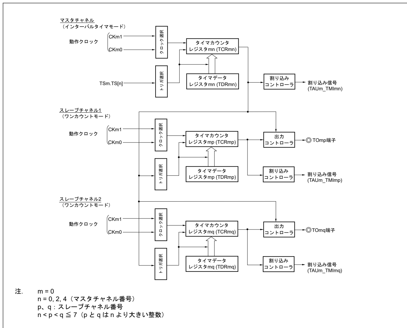
図 17.53 マルチ PWM 出力機能のブロック図 (2 種類の PWM 波形を出力する場合)
