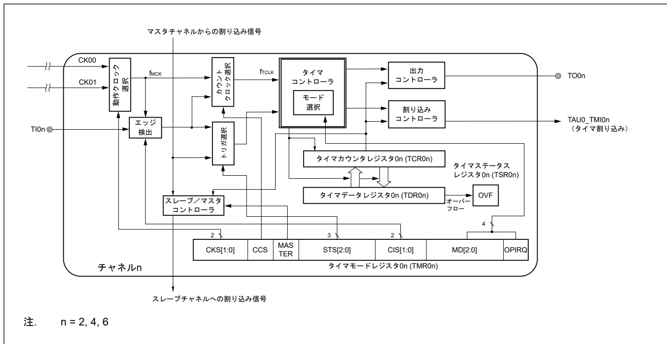
図 17.15 タイマアレiyユニット 0 のチャンネル 2、4、6 の内部ブロック図
