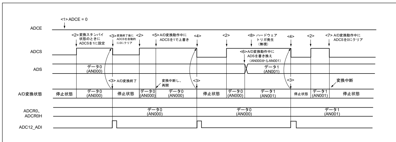
図 25.13 ソフトウェアトリガ待機モード（選択モード、ワンショット変換モード）動作タイミングの例
