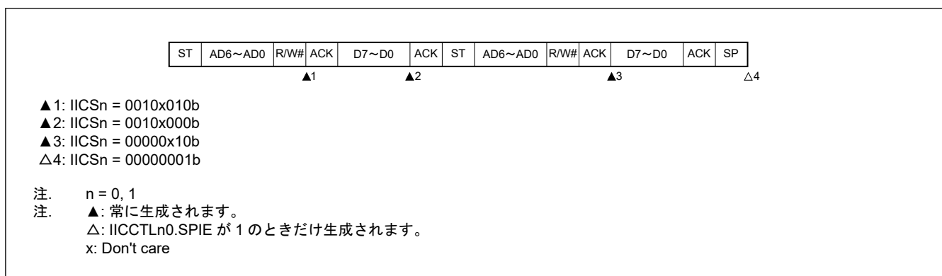
図 22.43 コードアクセスの後のスレーブデバイスの動作、一致しない (IICCTLn0.WTIM = 0)
