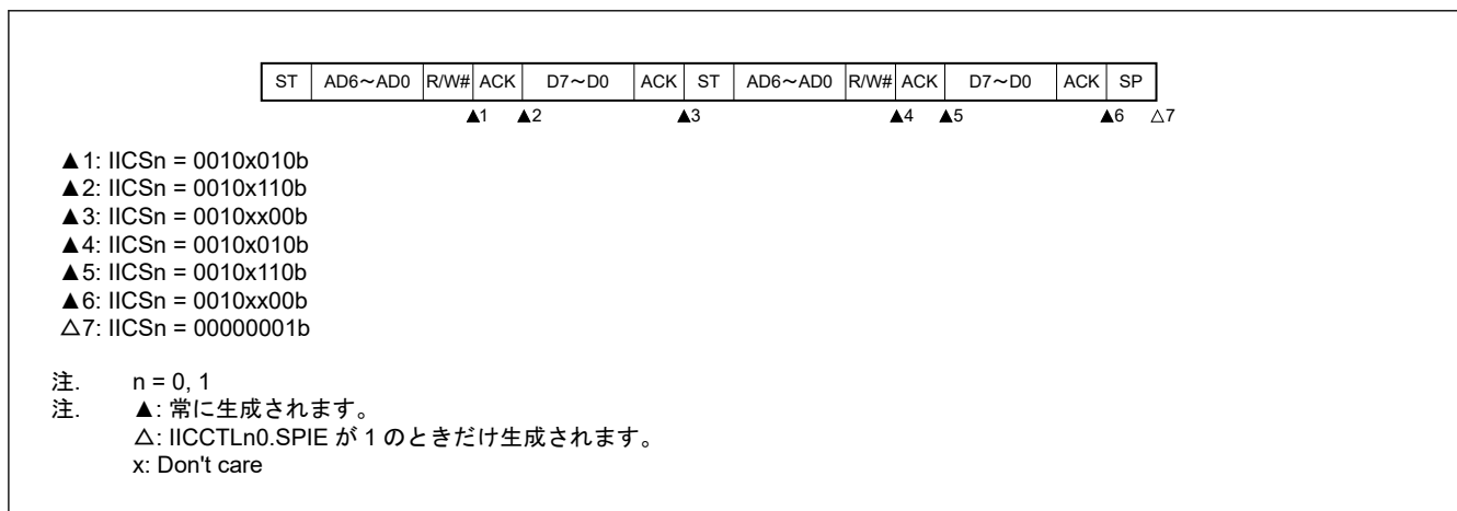
図 22.42 コードアクセスの後のスレーブデバイスの動作、拡張コードと一致する (IICCTLn0.WTIM = 1)
