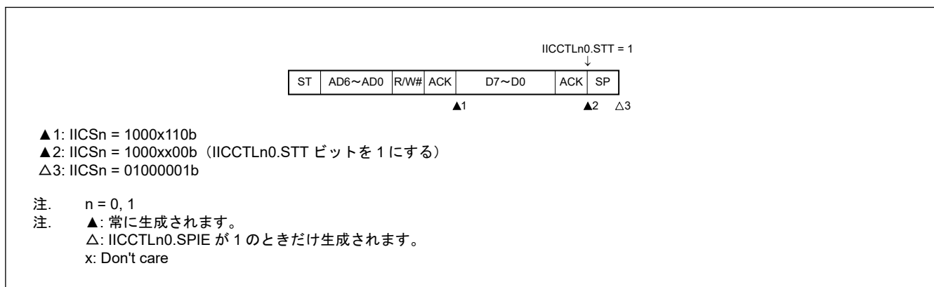
図 22.60 リスタートコンディションの生成を試みた時にストップコンディションによりアービトレーションロストが発生した場合の動作 (IICCTLn0.WTIM = 1)
