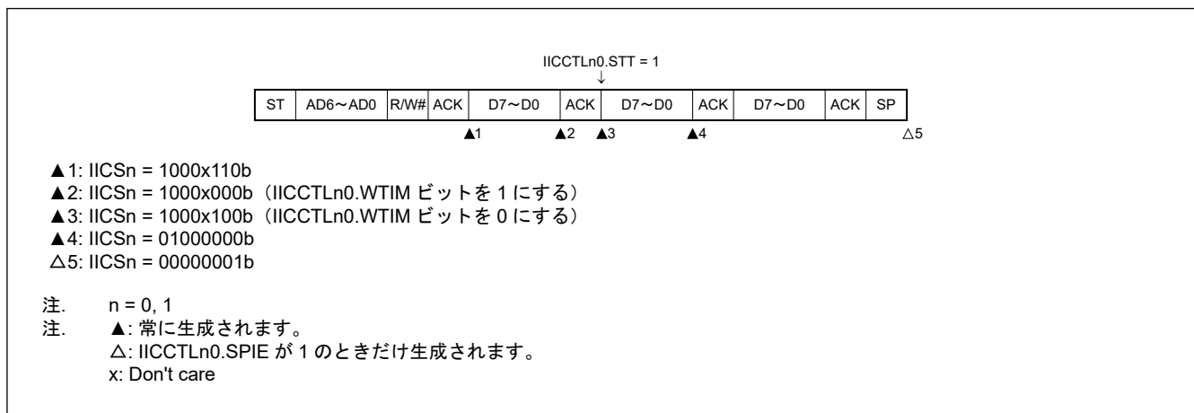
図 22.57 リスタートコンディションの生成を試みた時に Low レベルデータによりアービトレーションロストが発生した場合の動作 (IICCTLn0.WTIM = 0)
