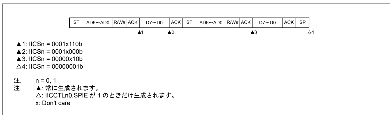
図 22.35 通常アクセスの後のスレーブデバイスの動作、一致しない (IICCTLn0.WTIM = 0)
