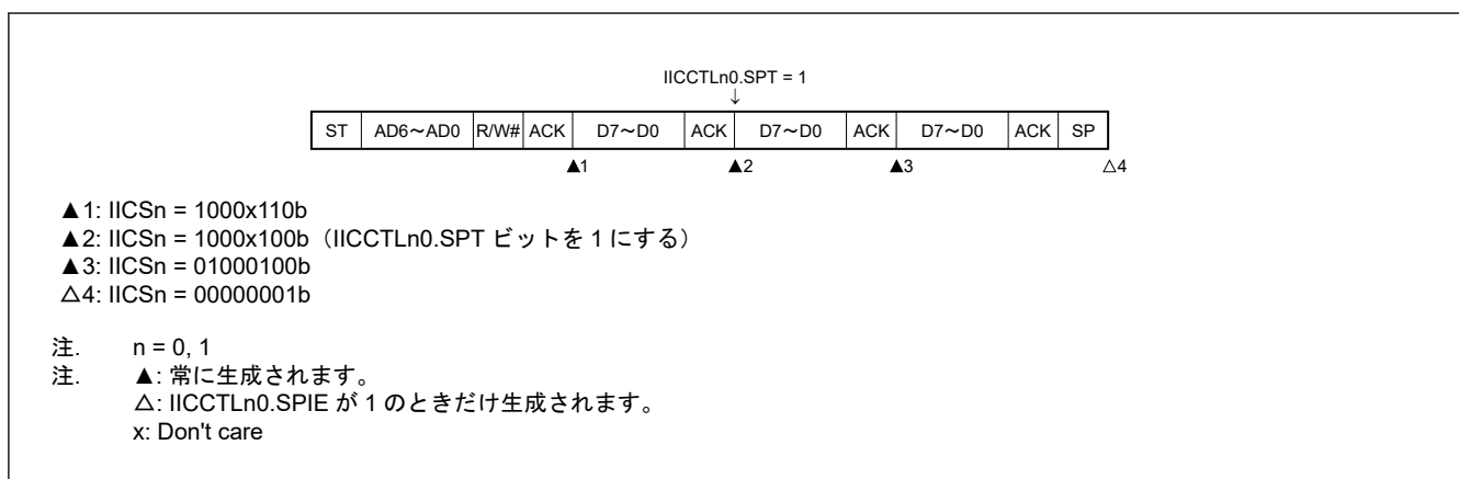
図 22.62 ストップコンディションを生成しようとしたときの S の Low レベルデータのためにアービトレーションロストが発生した場合の動作 (IICCTLn0.WTIM = 1)
