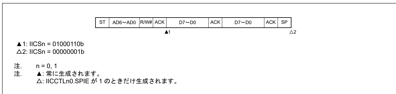
図 22.50 スレーブアドレスデータ送信時にアービトレーションロストが発生した場合の動作（IICCTLn0.WTIM が 1 の場合）
