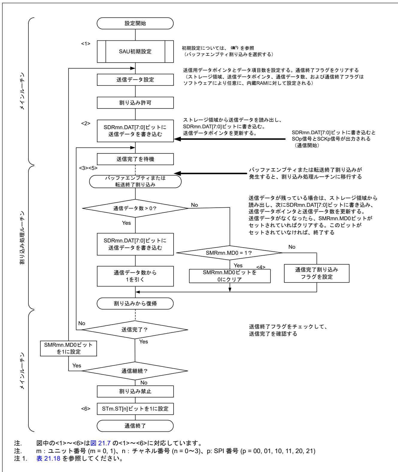
図 21.8 マスタ送信のフローチャート (連続送信モード時)
