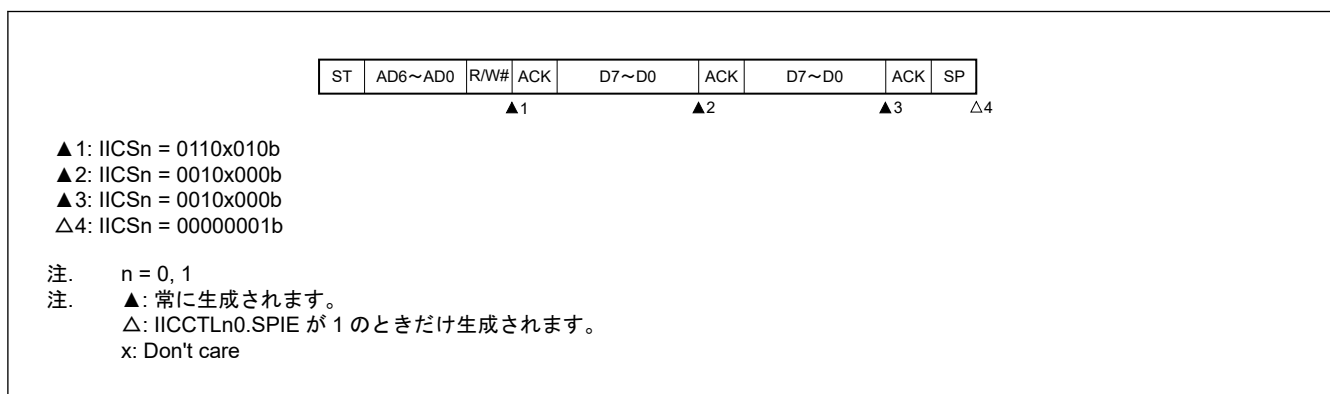
図 22.48 拡張コード送信時のアービトレーションロスト（IICCTLn0.WTIM が 0 の場合）
