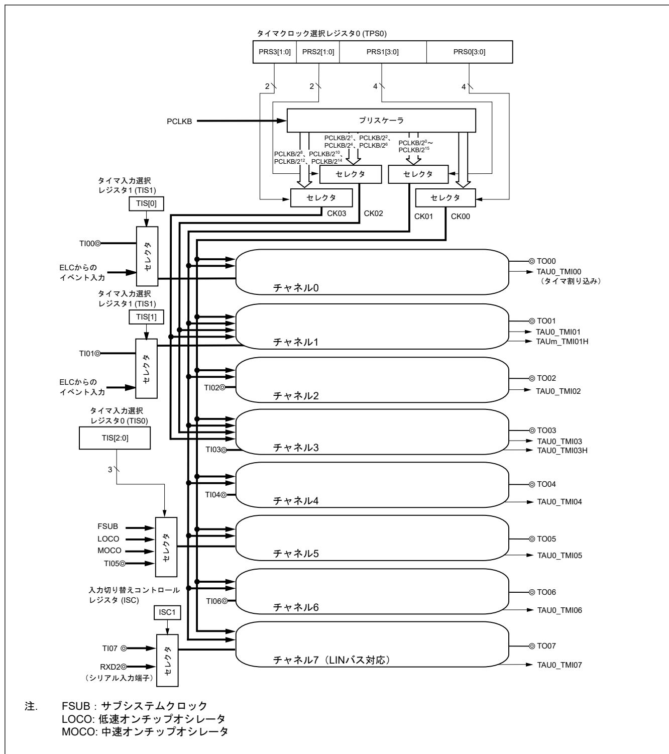
図 17.12 タイマアレiyユニット 0 の全体構成
