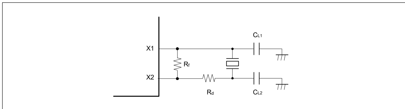
図 8.3 発振子の接続例
