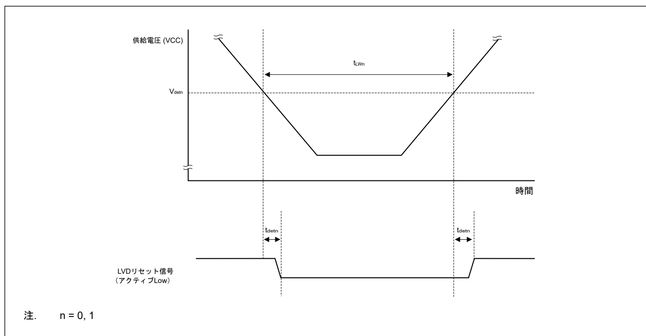
図 31.35 電圧検出回路タイミング
