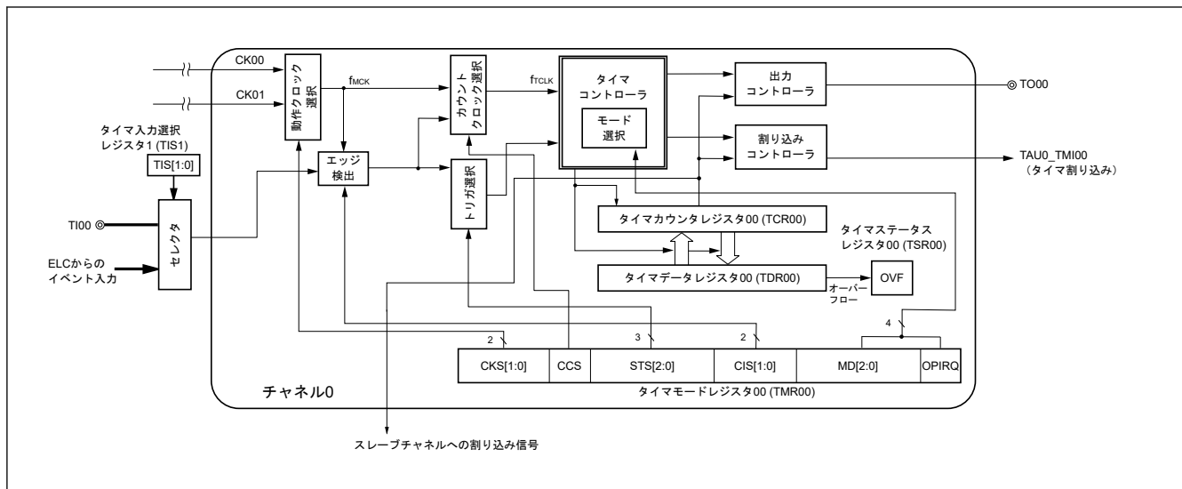
図 17.13 タイマアレユニット 0 のチャンネル 0 の内部ブロック図
