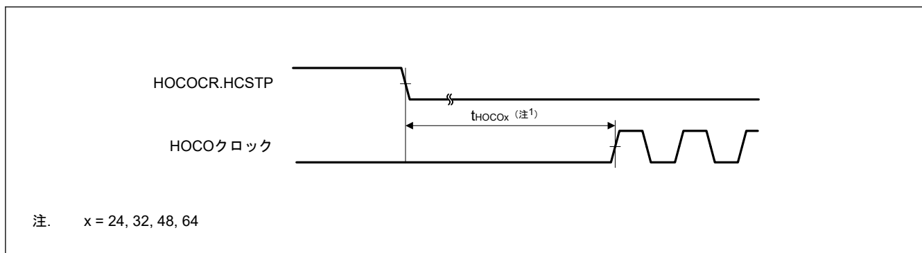
図 35.5 HOCO クロック発振開始タイミング (HOCOx.HCSTP ビット設定により開始)
