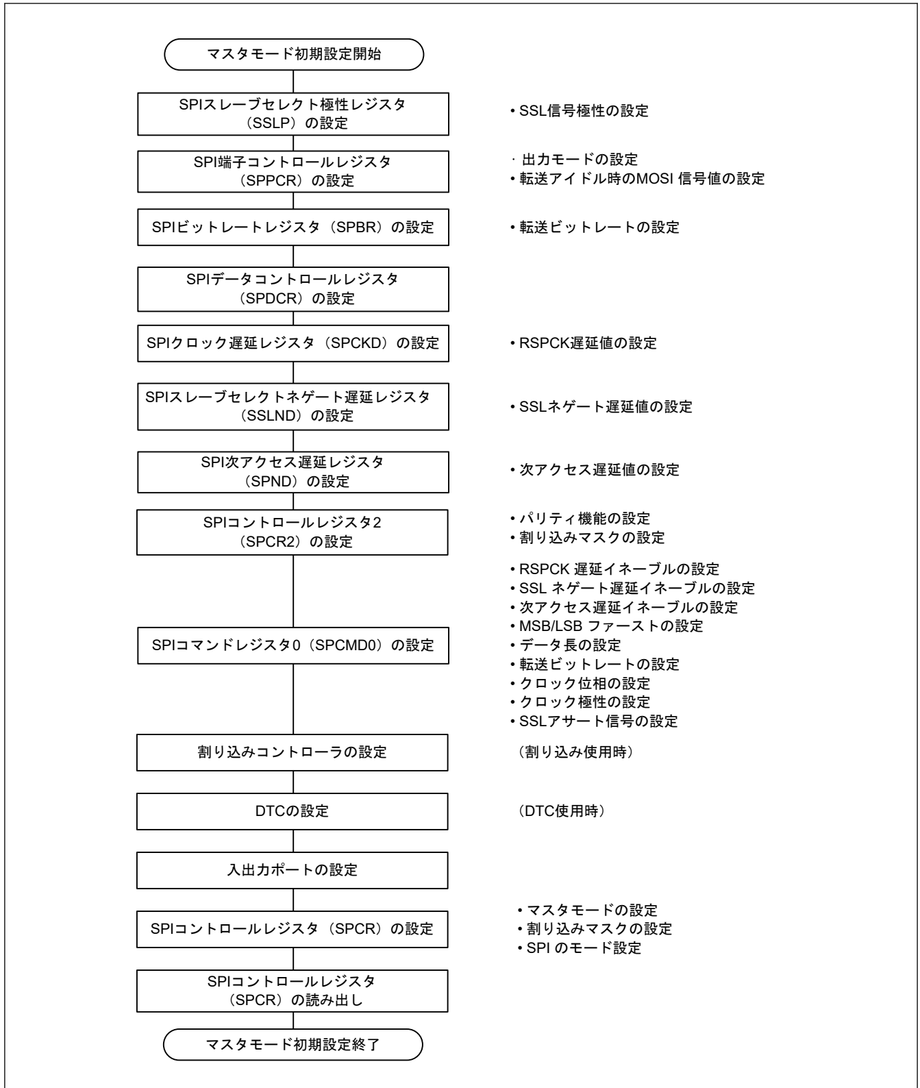
図 27.31 マスタモード時の SPI 動作の初期化フロー例
