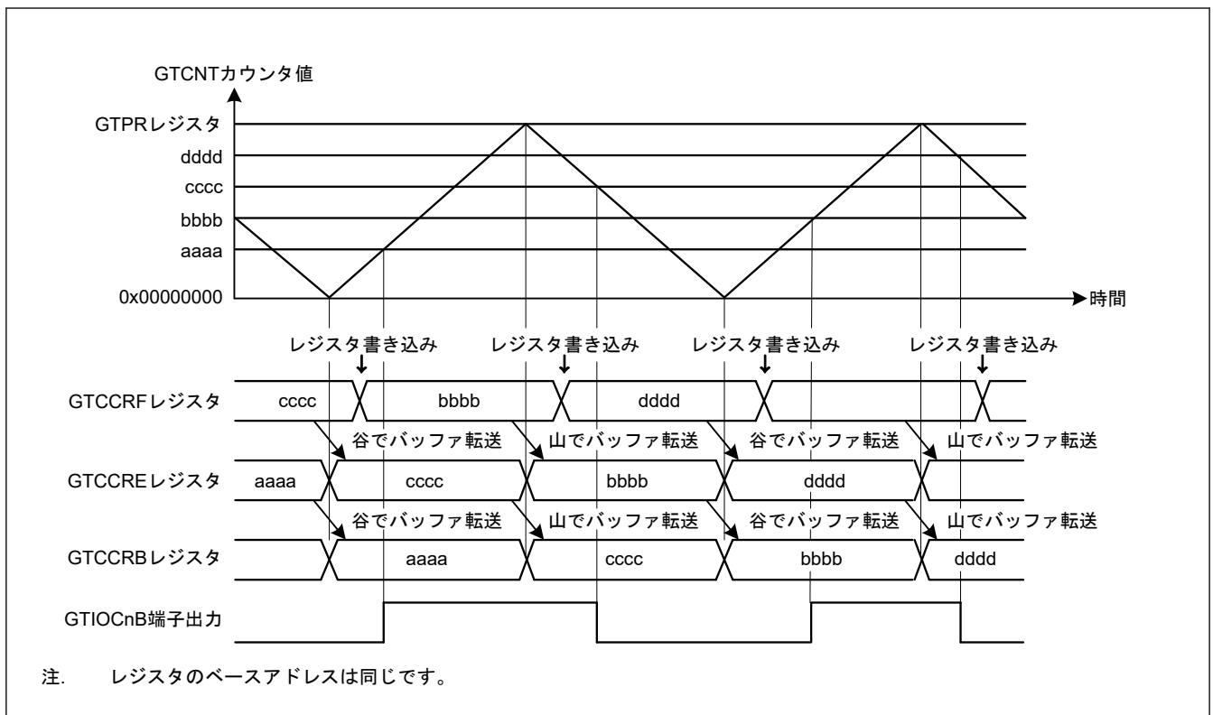
図 20.16 GTCCRA レジスタと GTCCRB レジスタのダブルバッファ動作例 (アウトプットコンペア、三角波、山と谷でバッファ動作、GTCCRB レジスタのコンペアマッチでトグル出力、周期の終わりで出力保持の場合)
