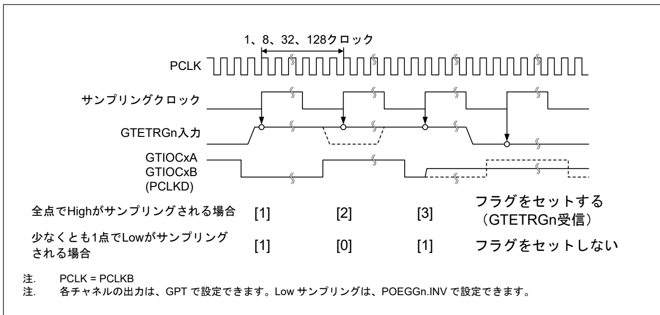
図 19.2 デジタルフィルタの動作例
