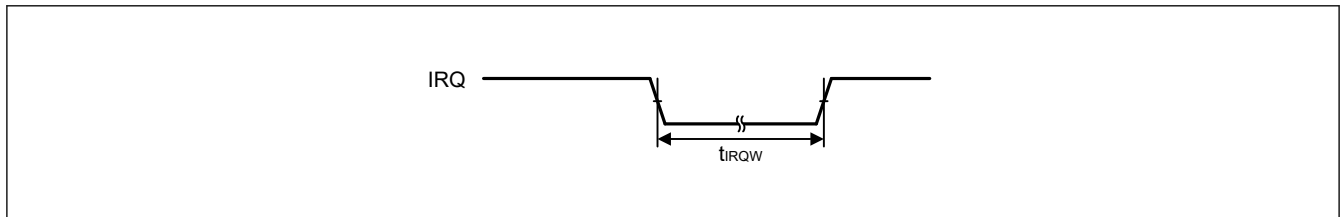
図 35.13 IRQ 割り込み入カタイミング
