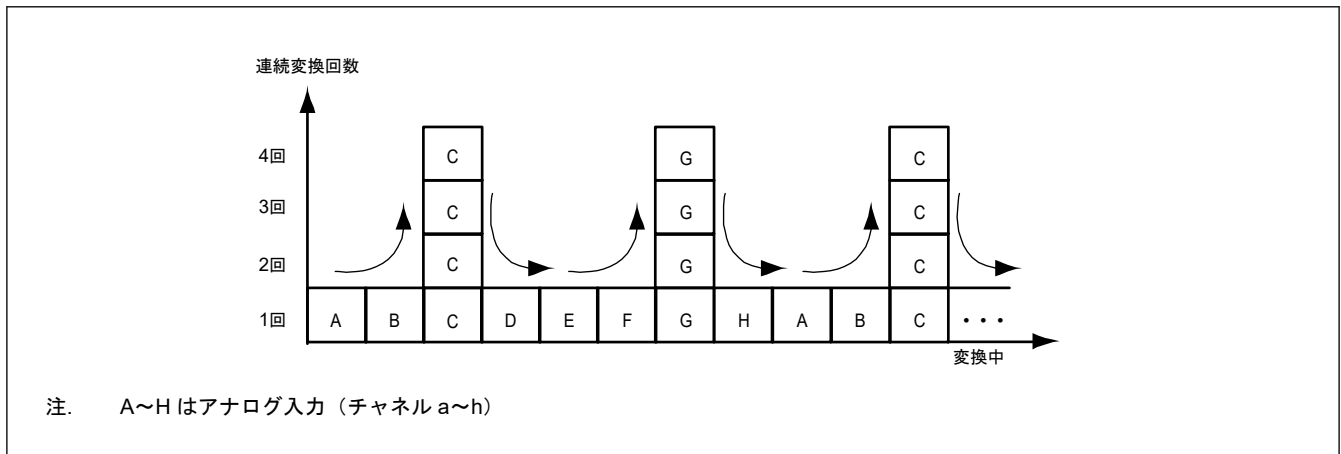
図 30.2 ADADC.ADC[2:0] = 011b および ADADS0/1 によるアナログ入力 C と G を 1 に選択時のスキャン変換シーケンス
