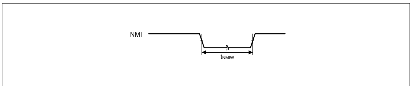
図 41.12 NMI 割り込み入カタイミング
