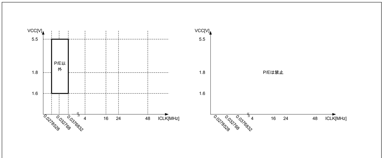
図 10.7 Subosc-speed モードにおける動作電圧と動作周波数
