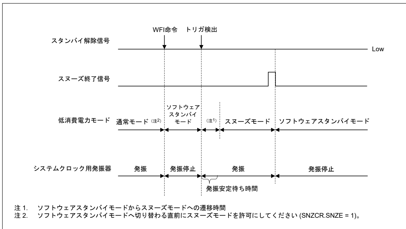
図 10.11 割り込み要求信号が発生しない場合のスヌーズモードの解除
