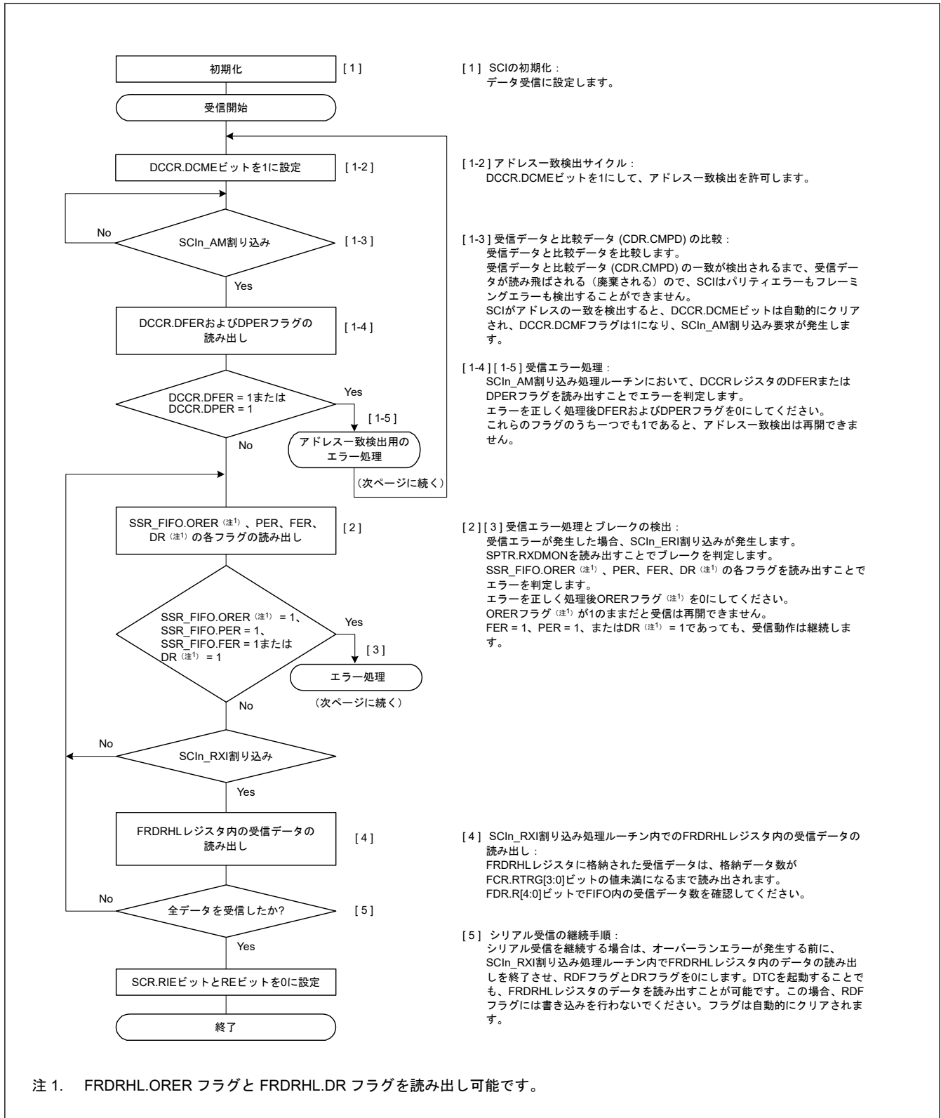
図 25.23 調歩同期式モードにおけるシリアル受信のフローチャート例 (FIFO 選択、アドレス一致検出有効時) (1)
