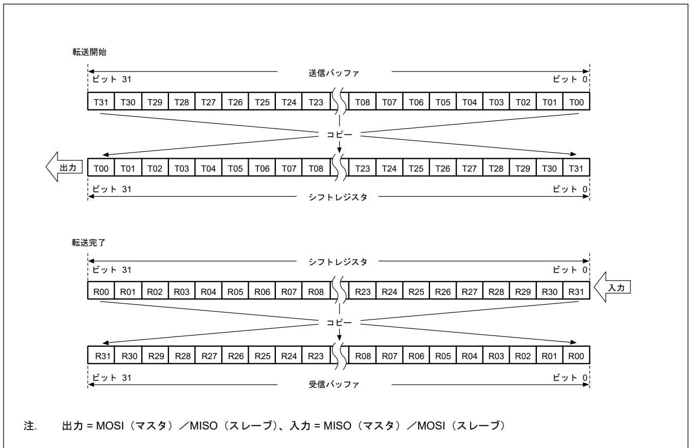
図 28.16 LSB ファースト転送 (32 ビットデータ/パリティ機能無効)
