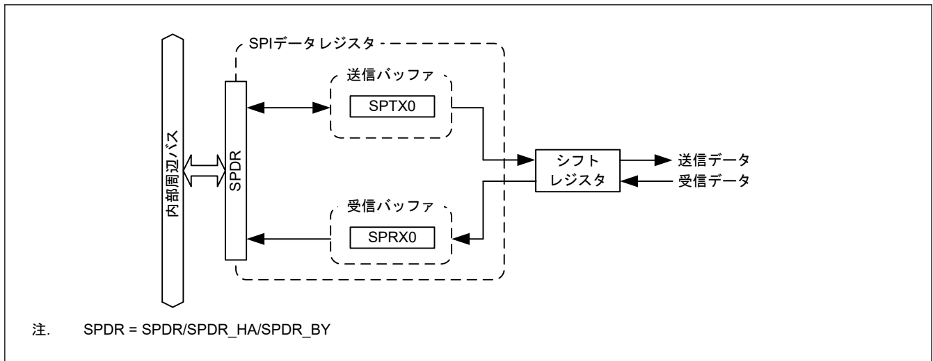
図 28.2 SPDR/SPDR_HA/SPDR_BY レジスタの構成図
