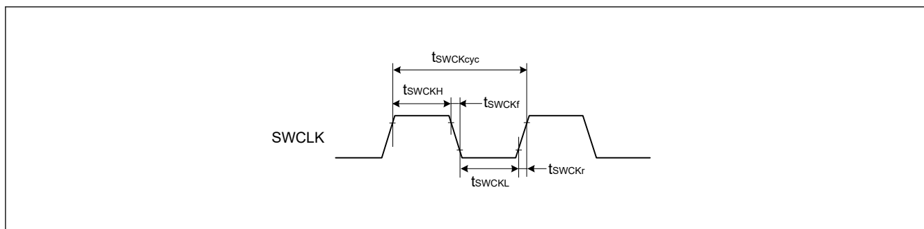
図 41.48 SWD SWCLK タイミング
