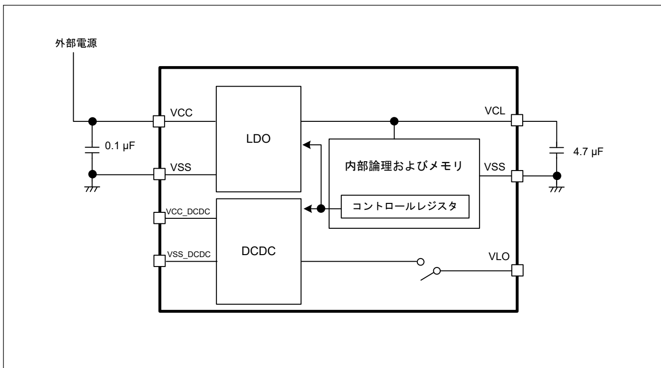
図 40.1 LDO の設定
