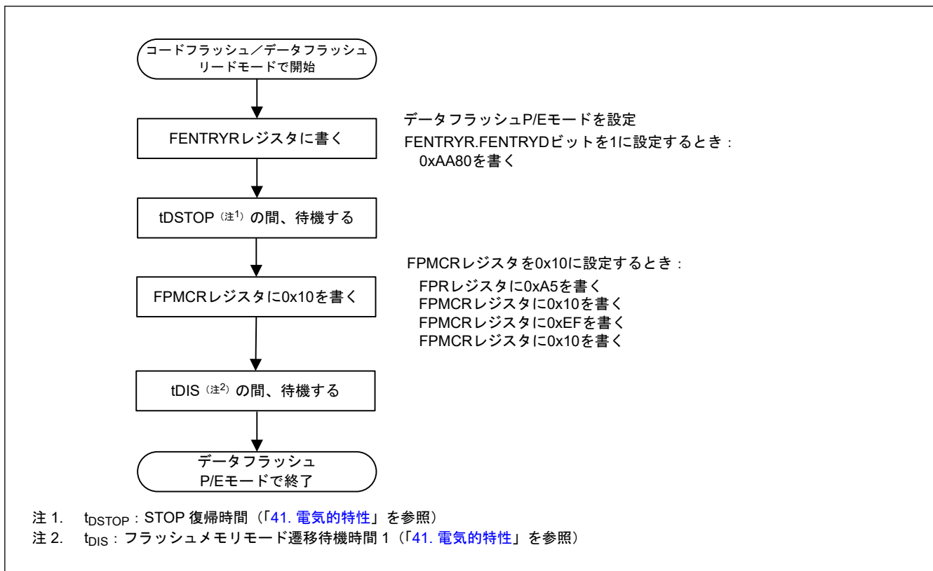
図 37.16 リードモードからデータフラッシュ P/E モードへの変更手順
