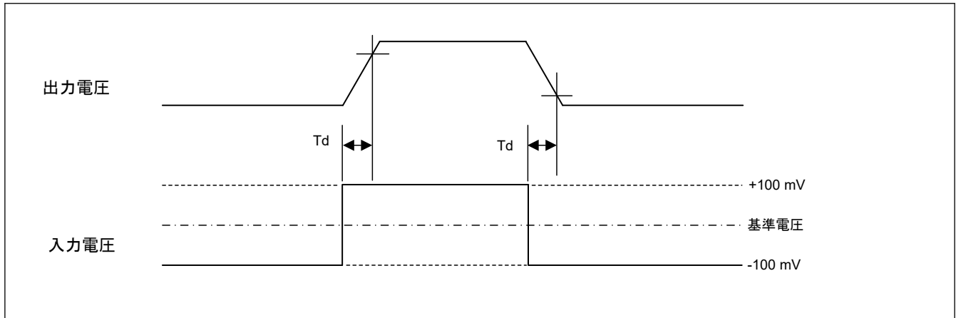
図 41.47 出力遅延時間
