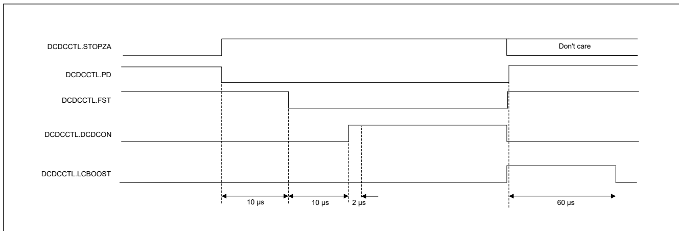
図 10.3 LDO 電源モード、DCDC 電源モード、Subosc-speed モード、ソフトウェアスタンバイモード間切り替え時の遷移タイミングとロード制限
