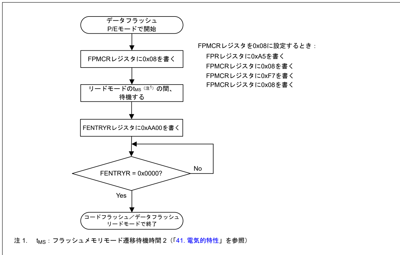
図 37.18 データフラッシュ P/E モードからリードモードへの変更手順
