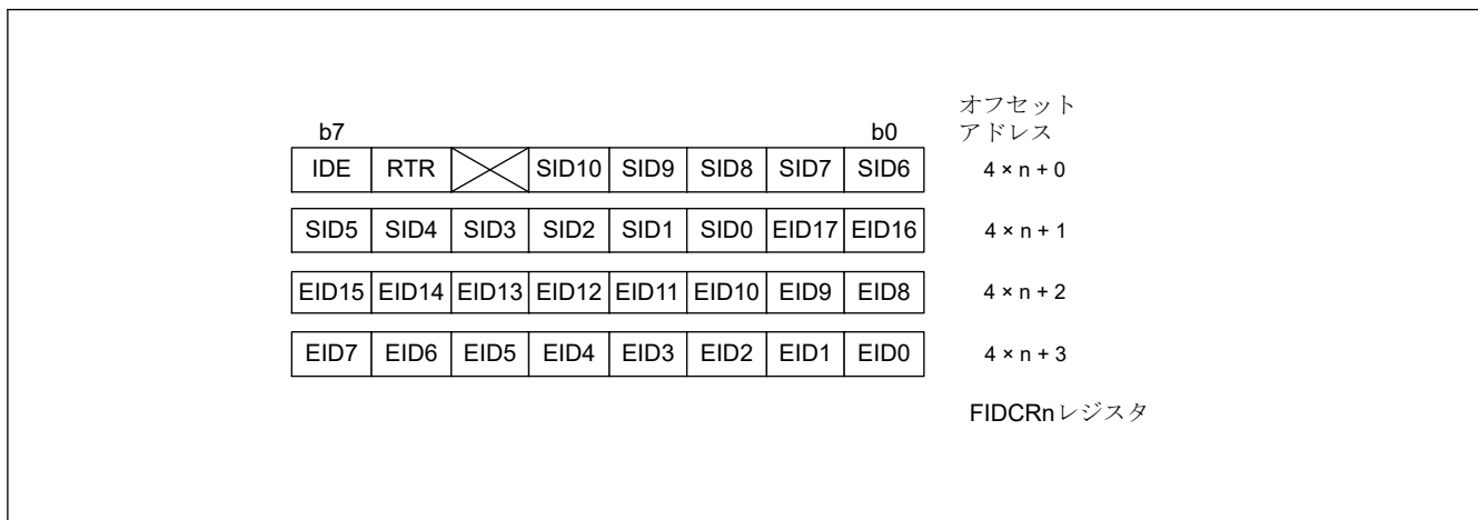
図 27.15 FIDCRn レジスタの構造 (n = 0)
