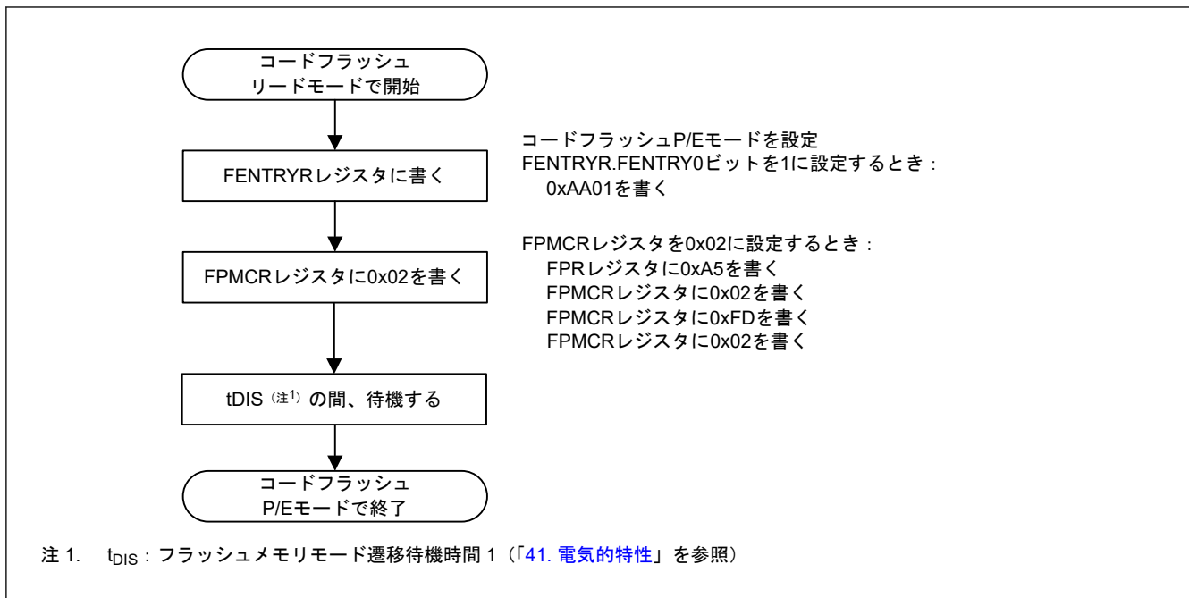
図 37.15 リードモードからコードフラッシュ P/E モードへの変更手順
