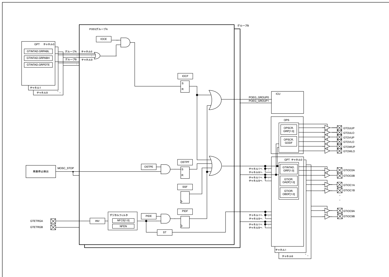
図 19.1 POEG のブロック図
