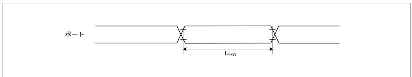
図 41.14 I/O ポート入力タイミング
