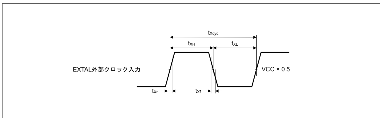
図 41.3 EXTERNAL クロック入力タイミング
