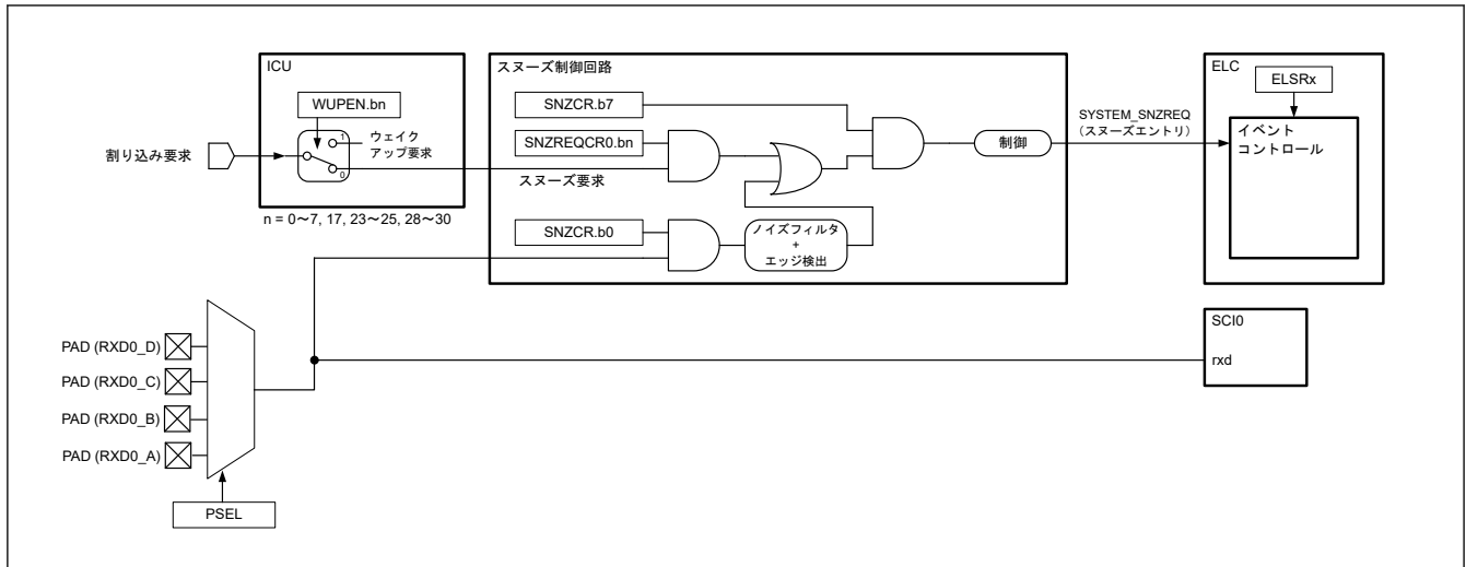
図 10.9 スヌーズモードエントリの構成
