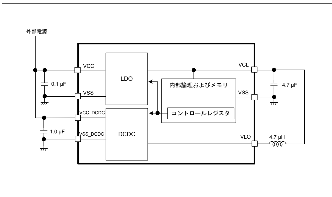
図 40.2 DCDC モード設定
