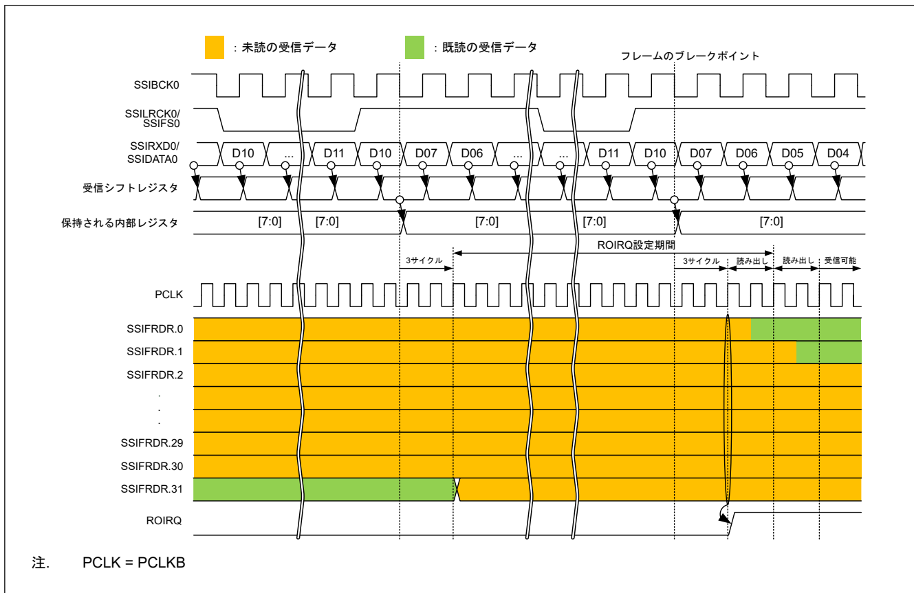
図 32.16 ROIRQ 設定タイミング
