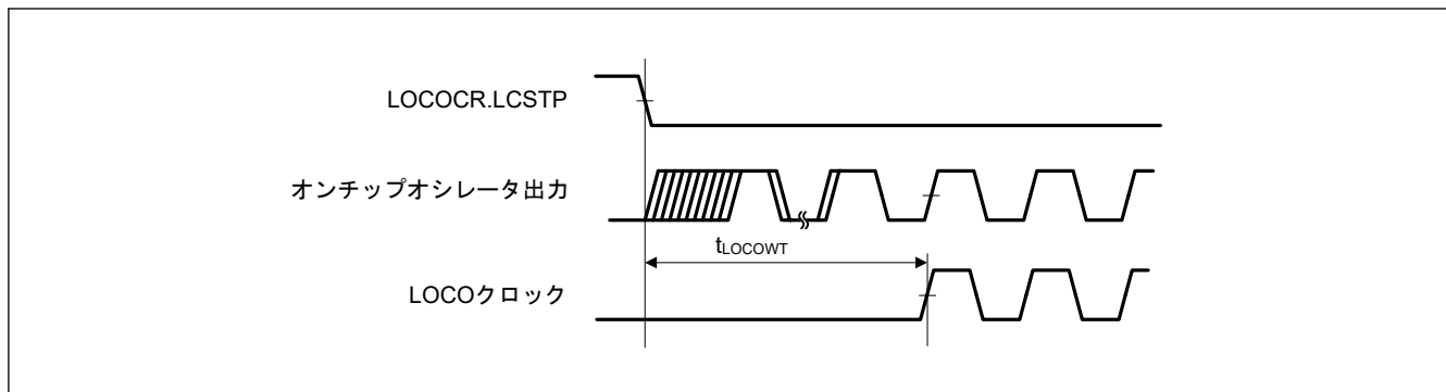
図 44.9 LOCO クロック発振開始タイミング
