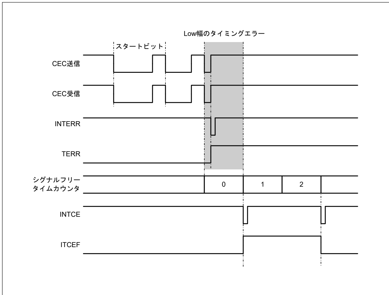
図 31.40 インシエータ動作時のタイミングエラー
