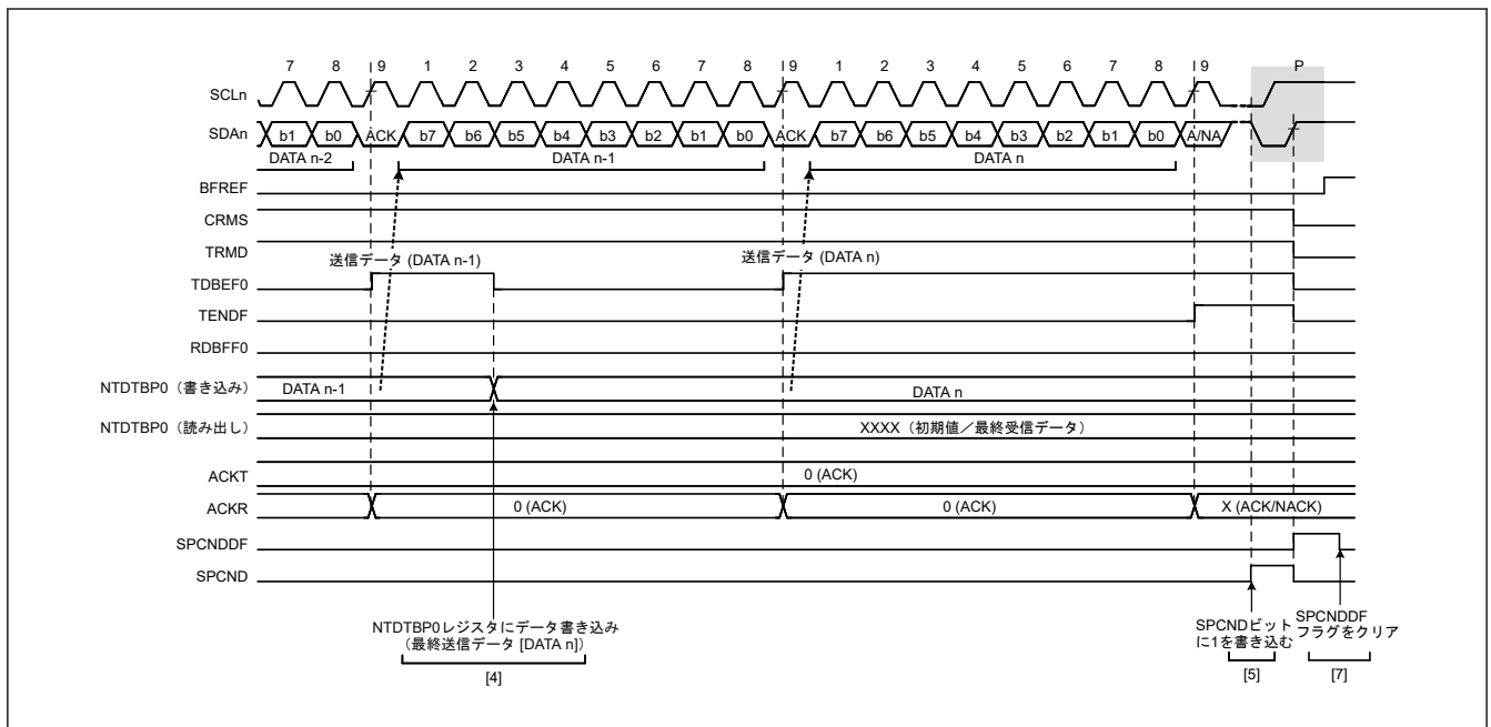
図 27.8 マスタ送信の動作タイミング (3)
