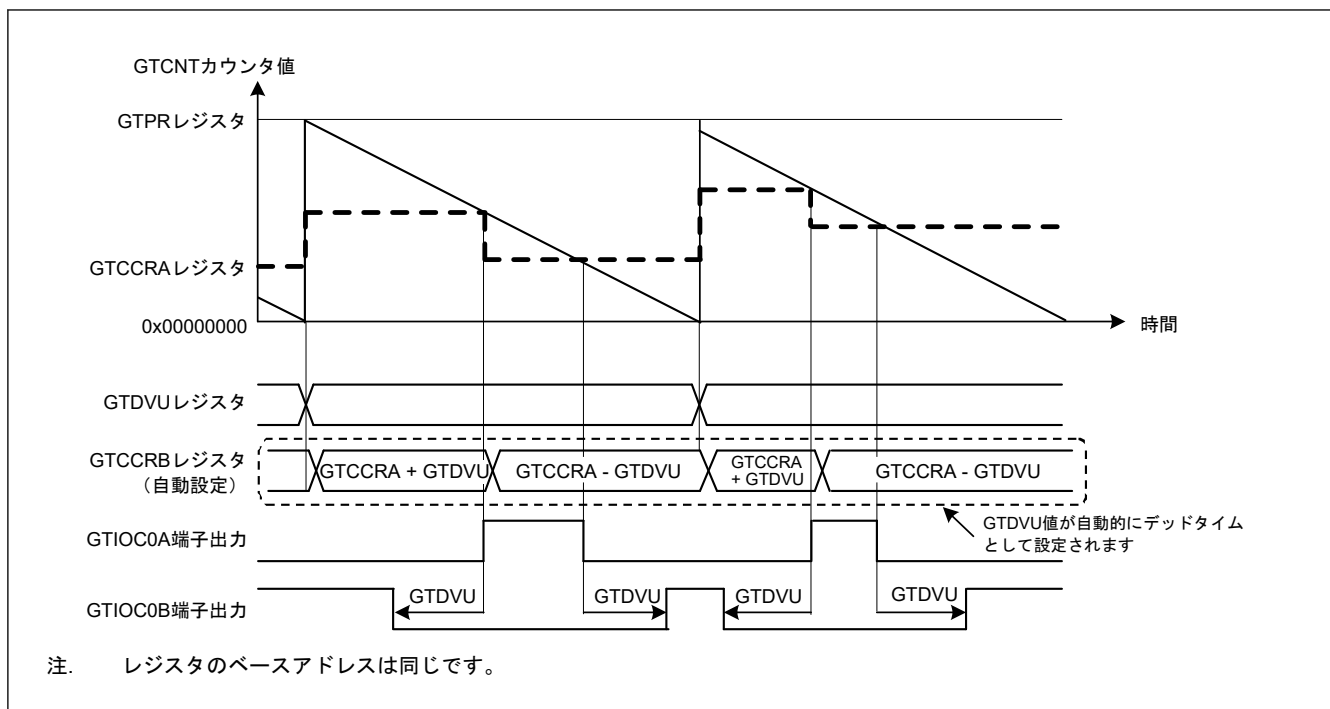
図 20.28 デッドタイム自動設定機能の動作例(のこぎり波ワンショットパルスモード、ダウンカウント、GTDVU/GTCCRB レジスタはバッファ動作、アクティブ High の場合)
