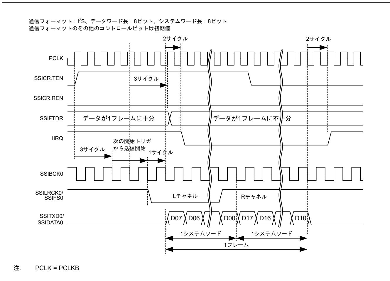
図 32.14 IIRQ 設定タイミング (送信)
