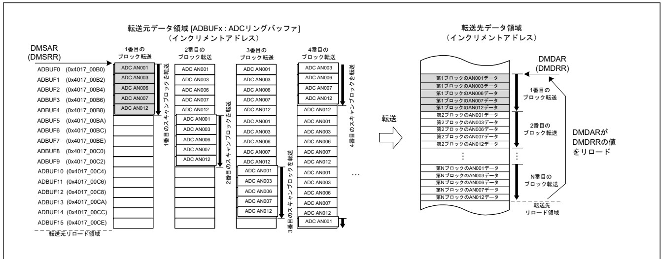
図 15.19 使用例：アラインされていないリングバッファからシングルリングバッファへ
