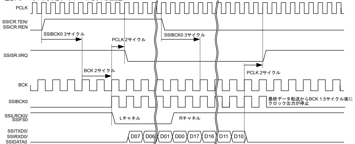
図 32.35 BCKASTP ビットの動作例 (BCKASTP = 1 での通信動作の場合)
