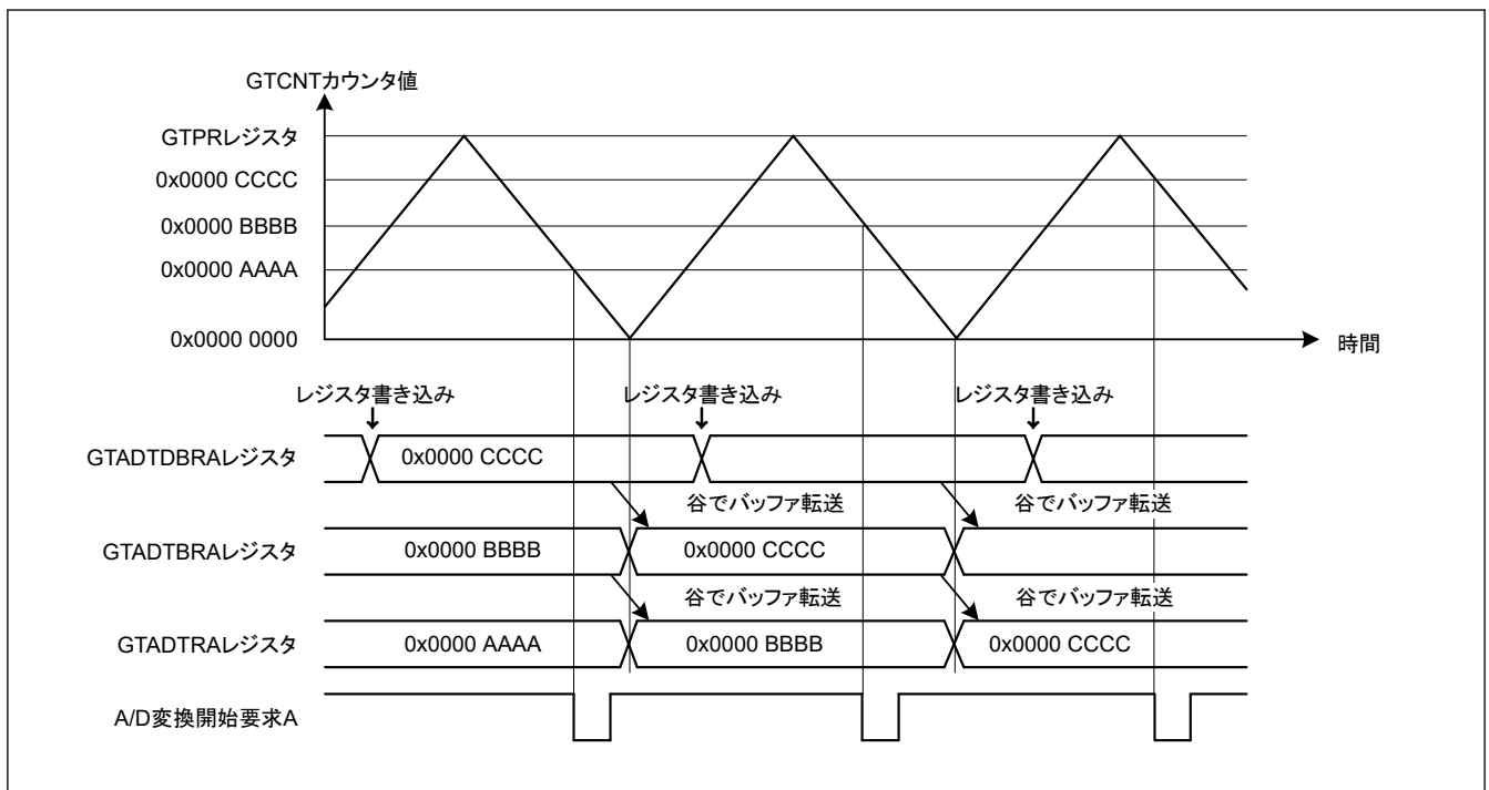
図 20.20 GTADTRA および GTADTRB レジスタのダブルバッファ動作例 (三角波、谷でバッファ転送、ダウンカウントで A/D 変換開始要求発生の場合)
