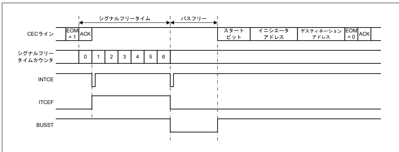
図 31.46 シグナルフリータイムの動作
