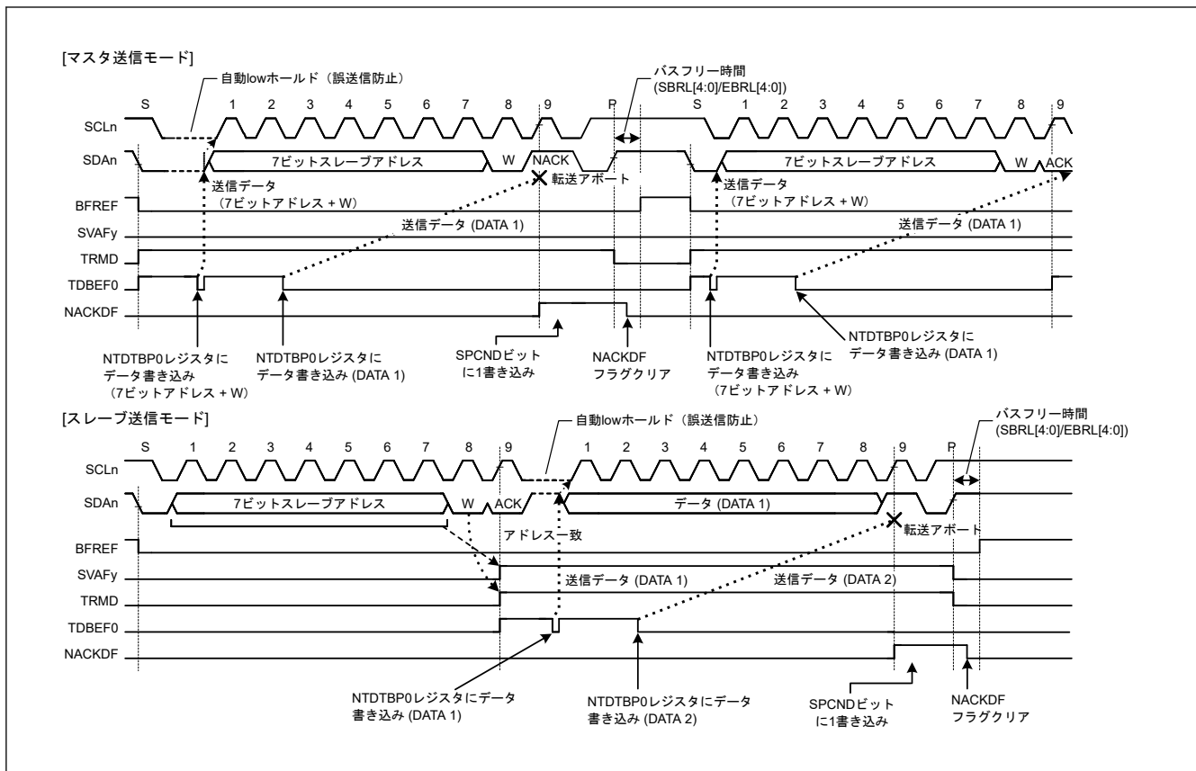
図 27.71 NACK 受信時のデータ転送中断動作 (NACKE = 1 の場合)
