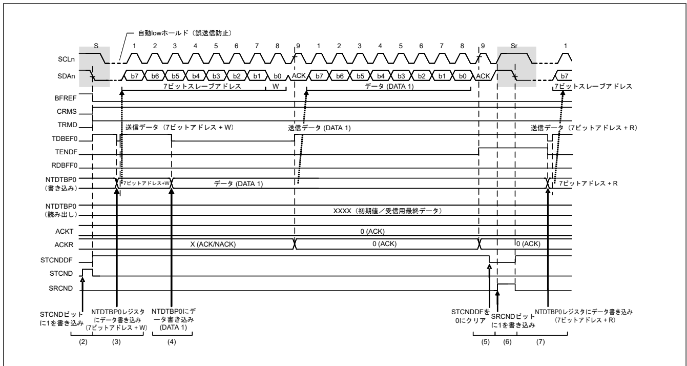
図 27.57 マスタ送信後の繰り返しのスタートコンディション発行タイミング
