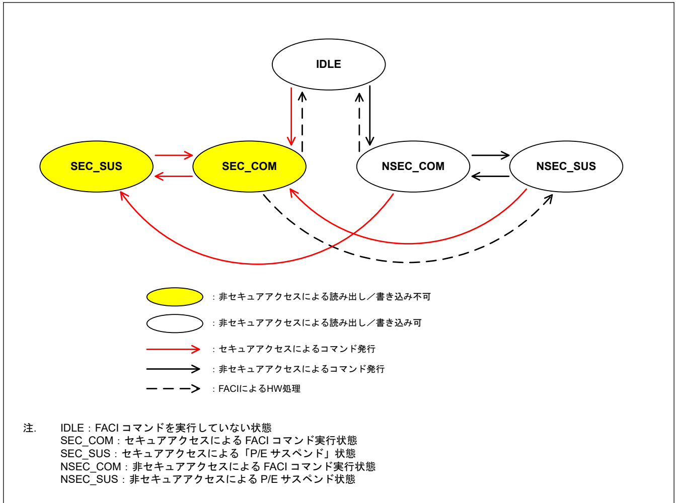
図 41.33 FACI コマンド動作中の保護状態
