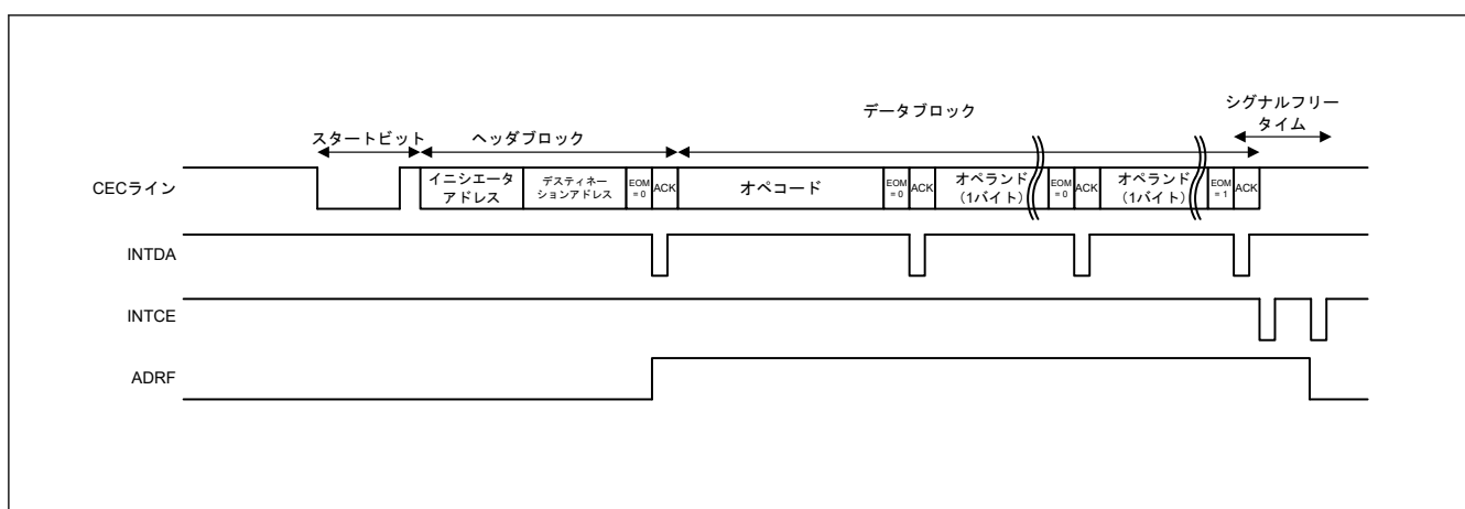
図 31.22 ADRF ビットの動作タイミング
