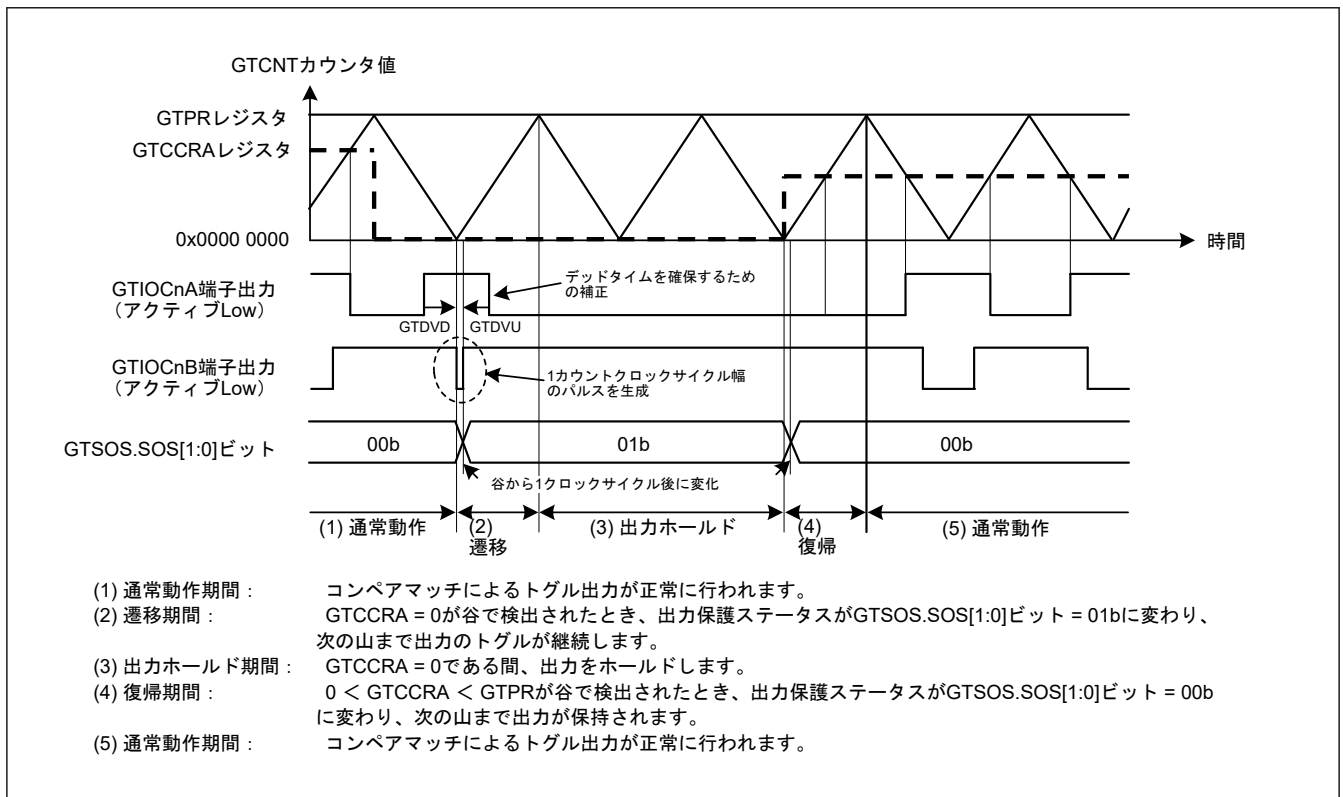
図 20.85 山でのパルファ転送中に GTCCRA が 0 になったときの出力保護機能の動作例 (谷でのパルファ転送中に 0 < GTCCRA < GTPR に復帰、アクティブレベルは Low) (n = 0, 1, 4, 5)
