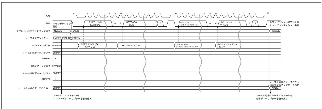
図 27.15 ダイナミックアドレス配置手順 (SETDASAs CCC) タイミング
