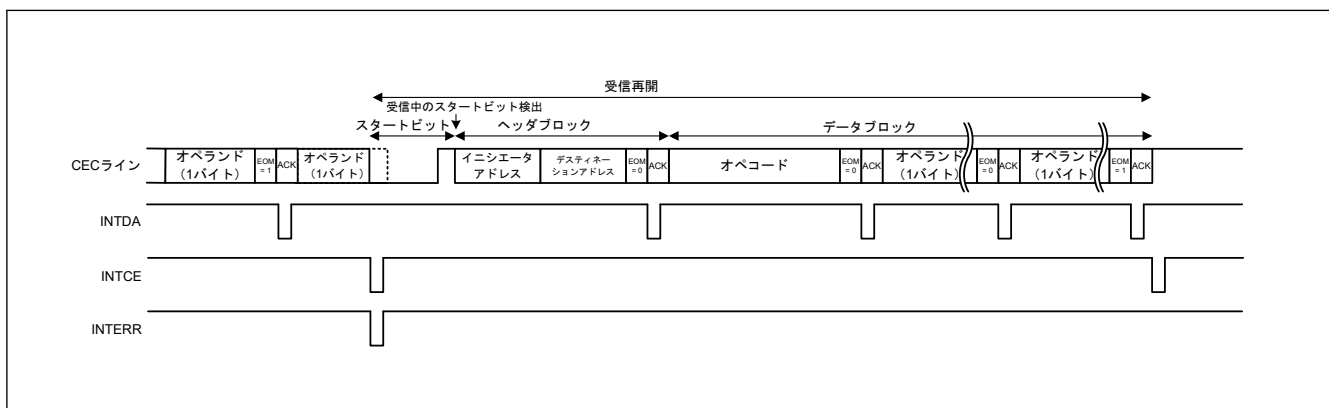
図 31.49 再受信機能動作
