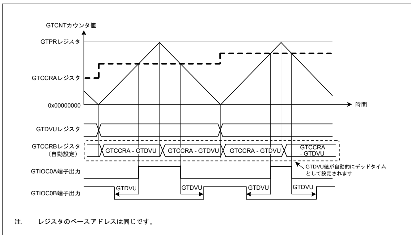
図 20.29 デッドタイム付きコンペアマッチ値の自動設定機能の動作例(三角波 PWM モード 1、GTDVU/GTCCRB レジスタはバッファ動作、アクティブ High の場合)
