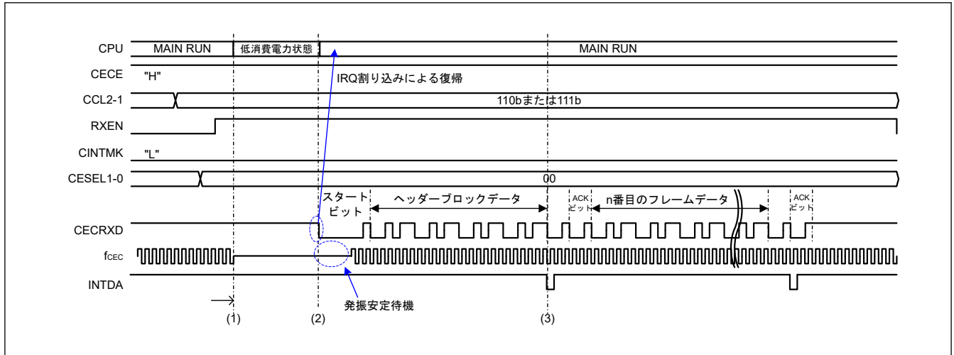
図 31.50 スタートビットの立ち下がリエッジによる低消費電力状態からの復帰動作
