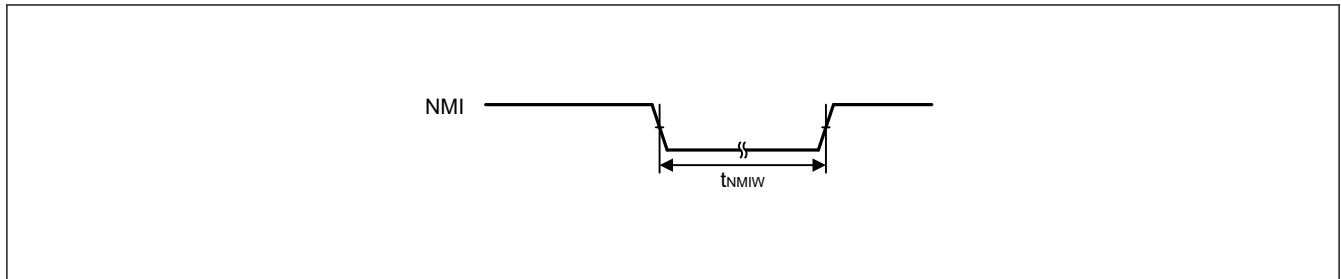
図 44.17 NMI 割り込み入カタイミング
