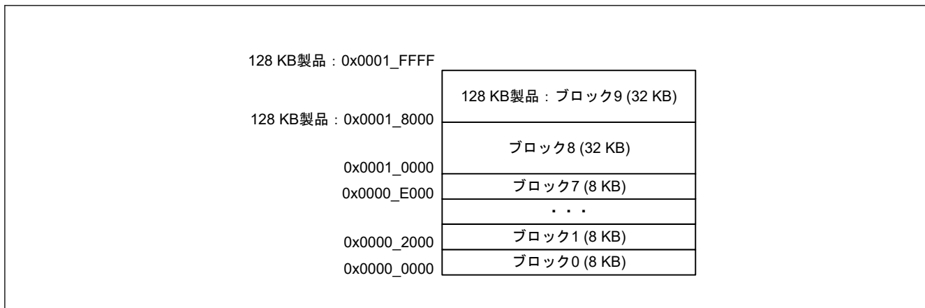
図 6.2 コードフラッシュのブロック構成
