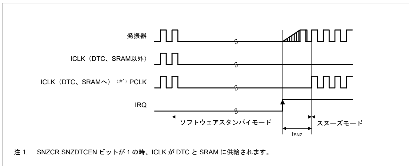
図 44.16 ソフトウェアスタンバイモードからスヌーズモードへの復帰タイミング
