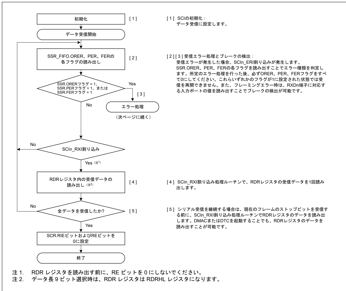
図 26.17 調歩同期式モードにおけるシリアル受信のフローチャート例（非 FIFO 選択、アドレス一致検出無効時）(1)
