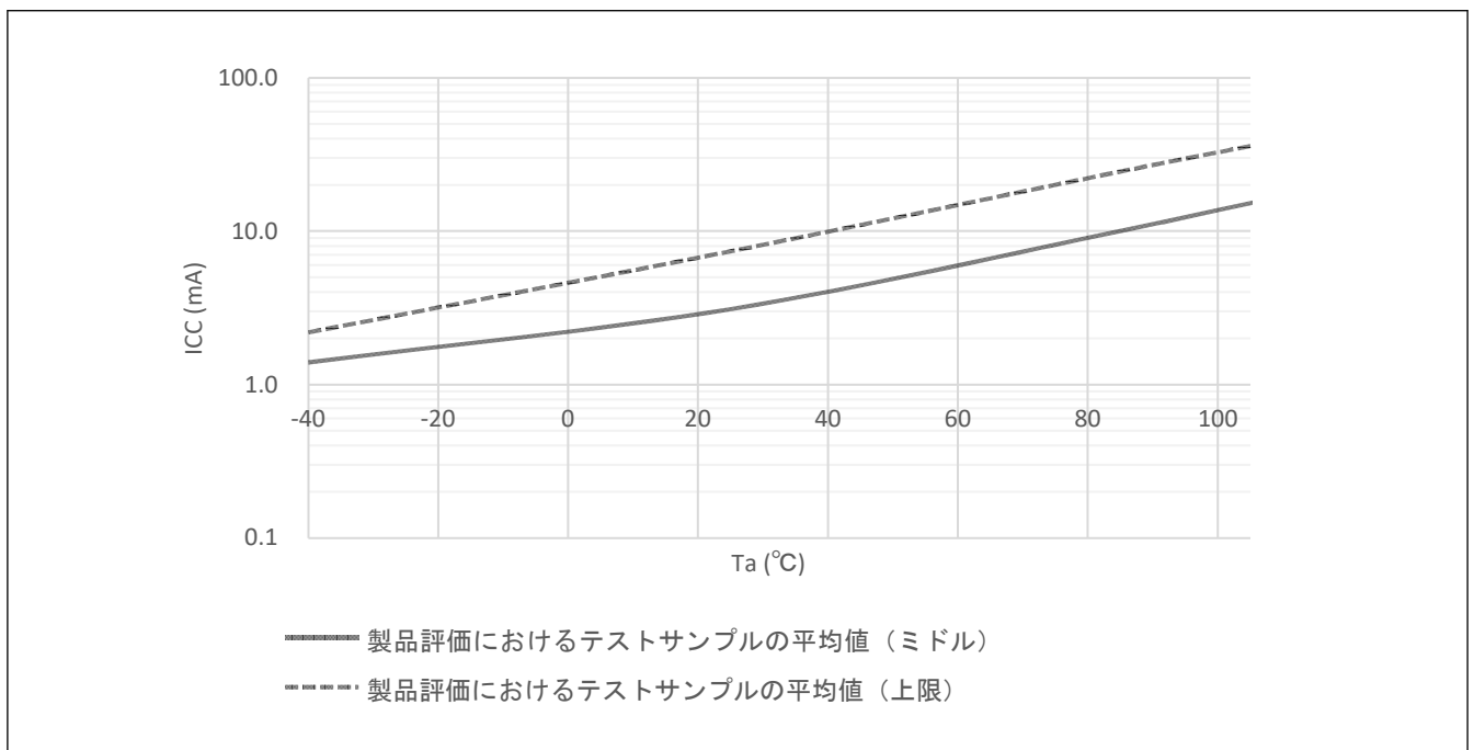
図 44.2 ソフトウェアスタンバイモード時の温度依存性 (参考データ)
