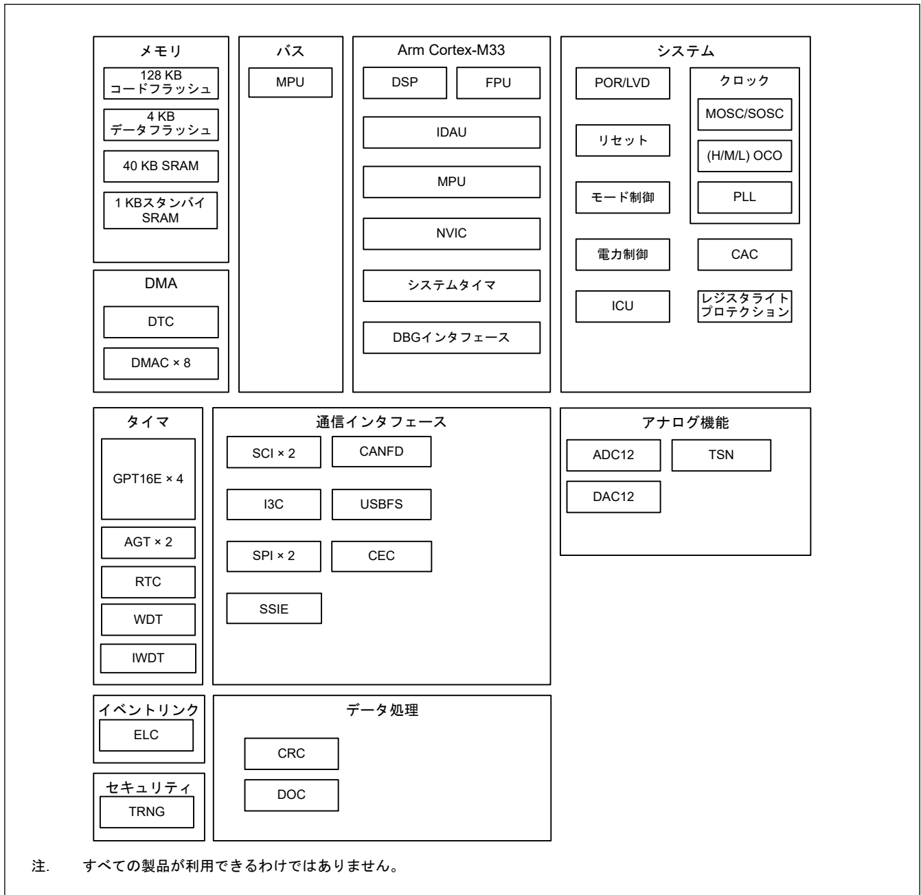
図 1.1 ブロック図
