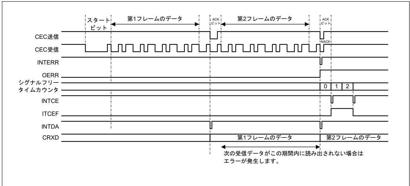
図 31.43 オーランエラー (シグナルフリータイム = 3 ビット幅設定時)
