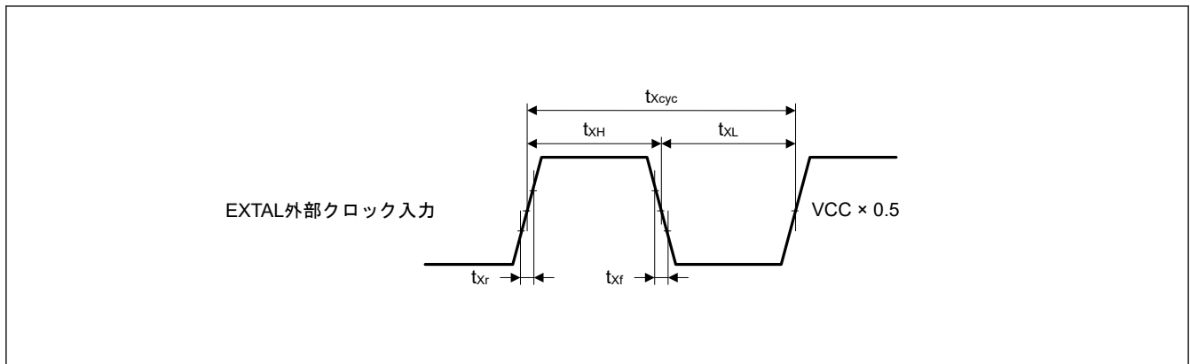
図 44.7 EXTERNAL 外部クロック入力タイミング
