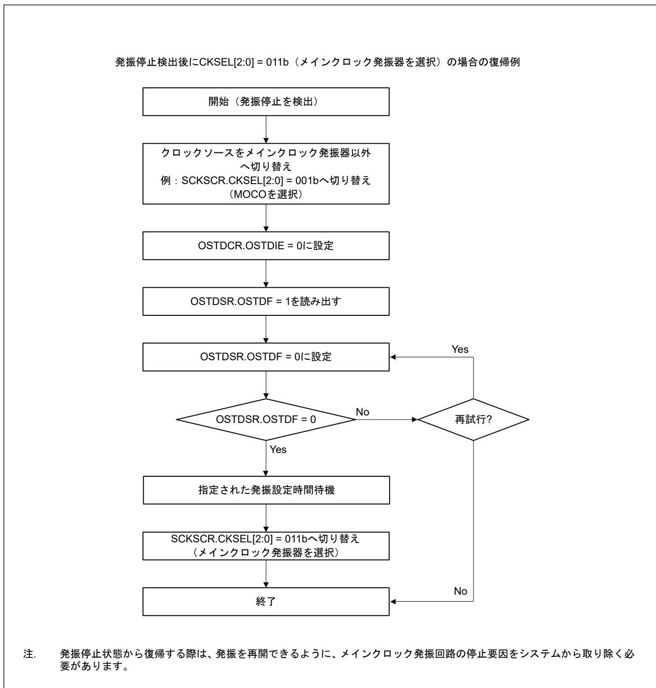
図 8.8 発振停止検出時の復帰フロー
