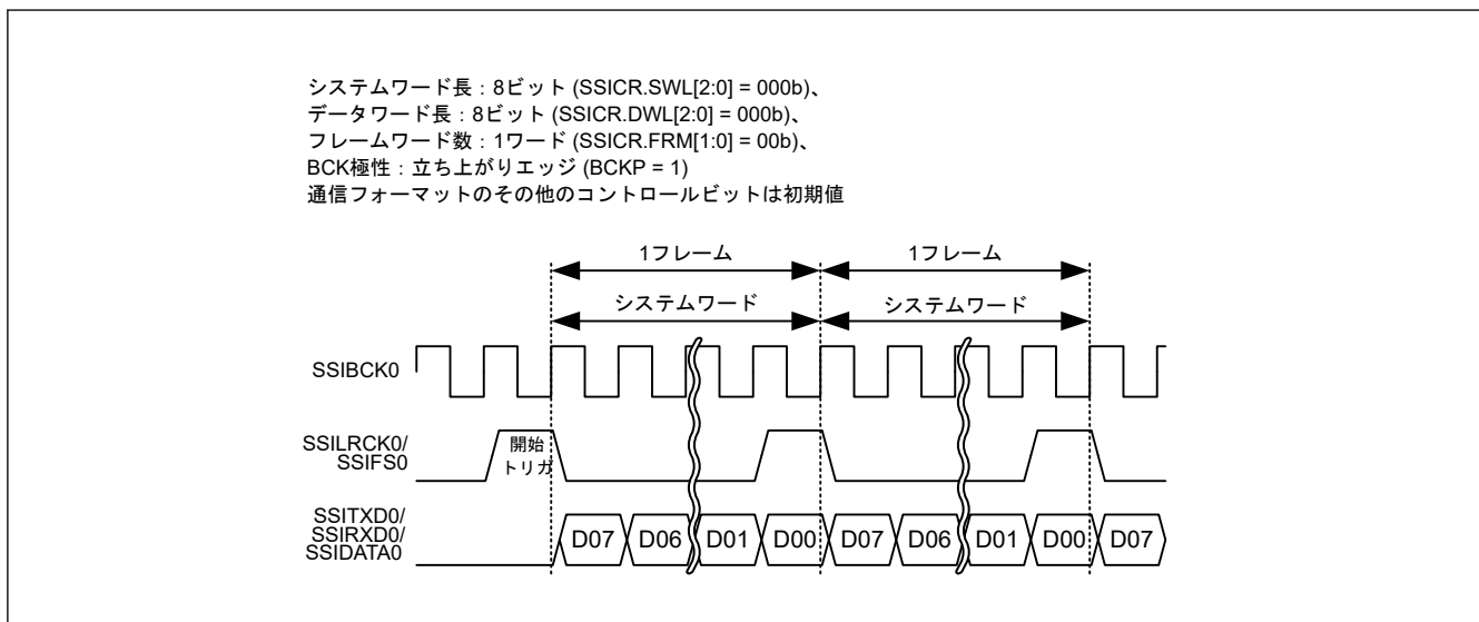
図 32.38 モノラルフォーマットにおけるショートフレーム (パディングなし、システムワード長 = データワード長)
