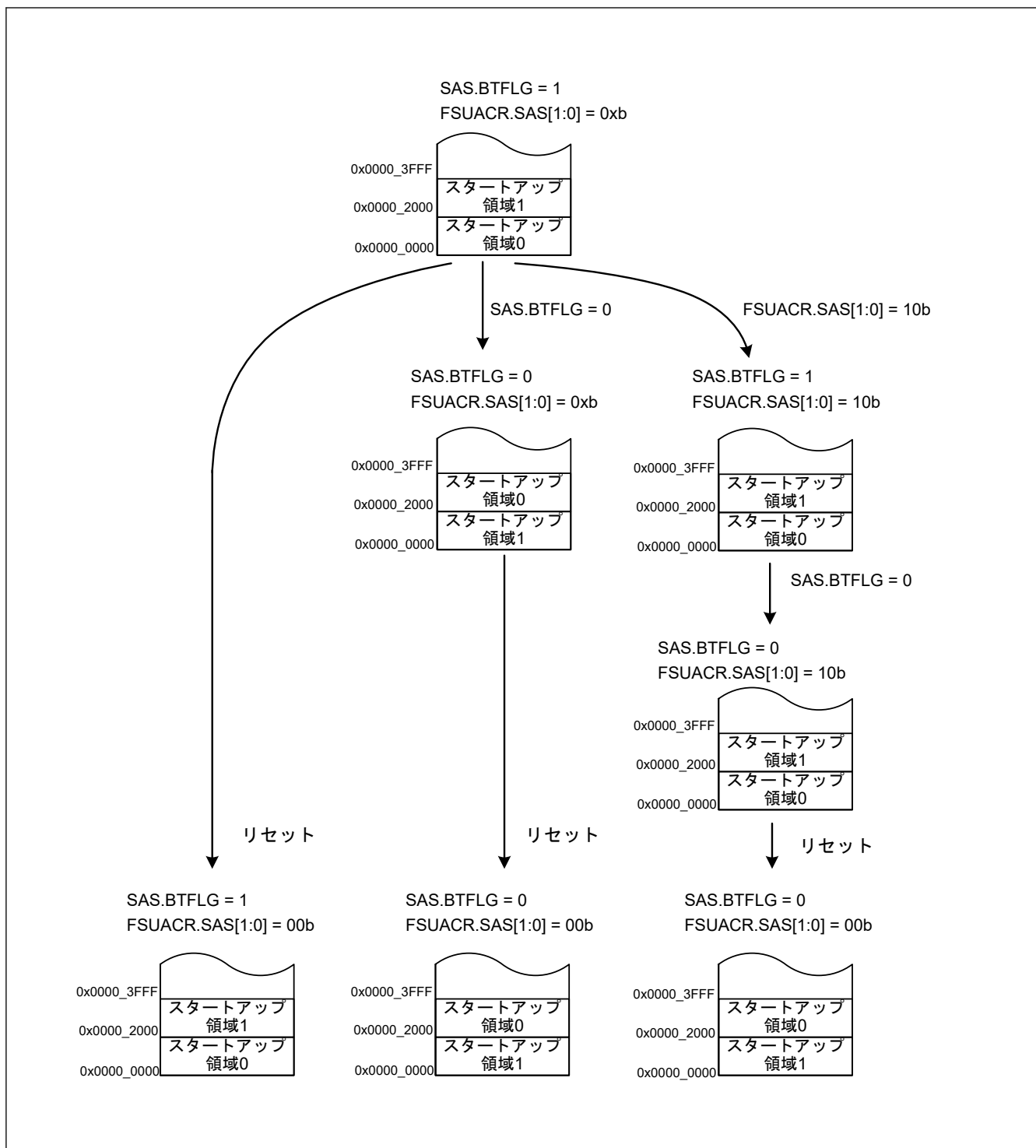
図 41.26 スタートアッププログラム保護設定の遷移例 1
