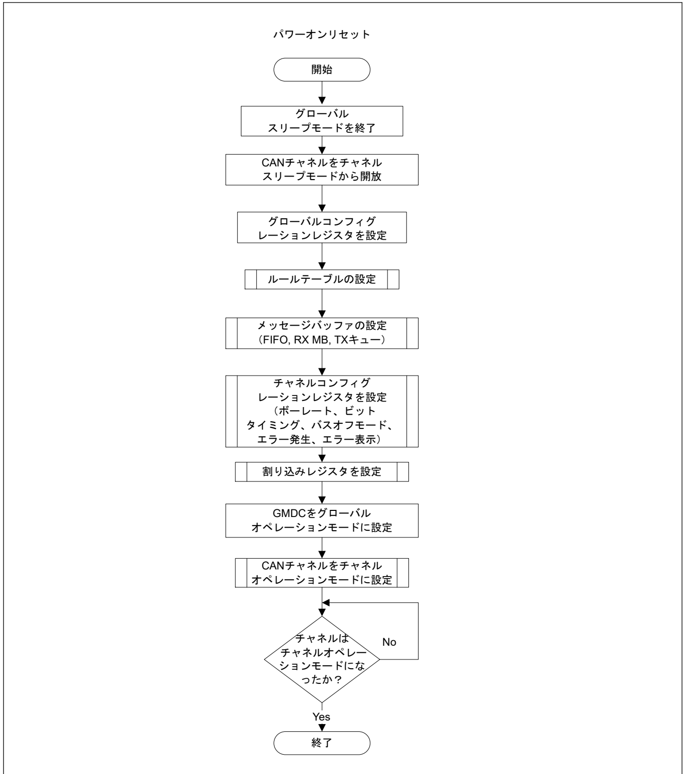
図 28.23 ハードウェアリセット後の構成手順
