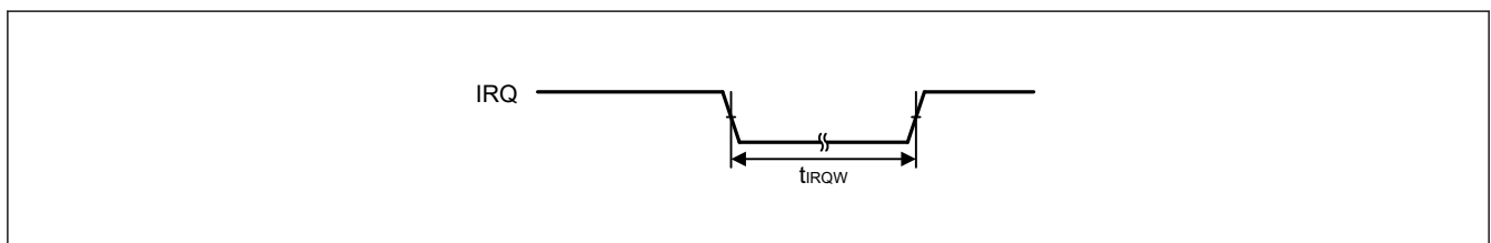
図 44.18 IRQ 割り込み入カタイミング
