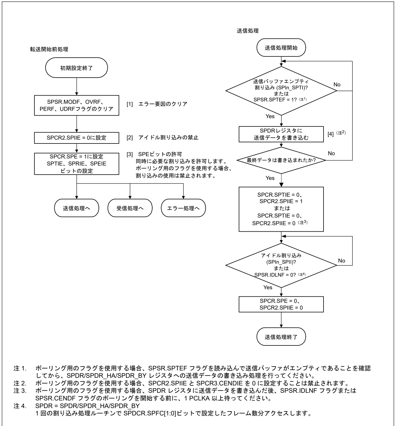
図 30.49 マスタモードでの送信フロー
