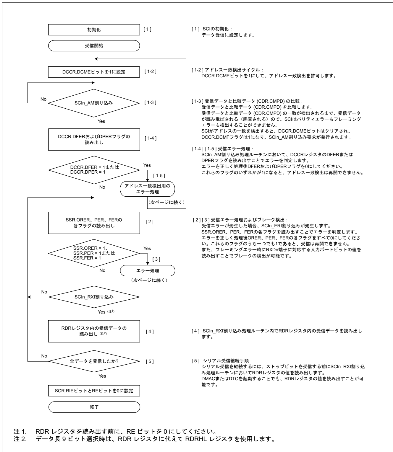
図 26.19 調歩同期式モードにおけるシリアル受信のフローチャート例（非 FIFO 選択、アドレス一致検出有効時）(1)
