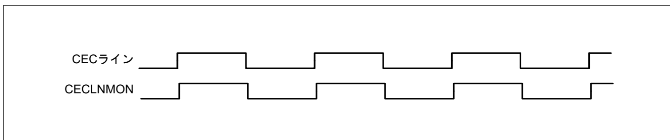
図 31.31 CECLNMON ビットのタイミング
