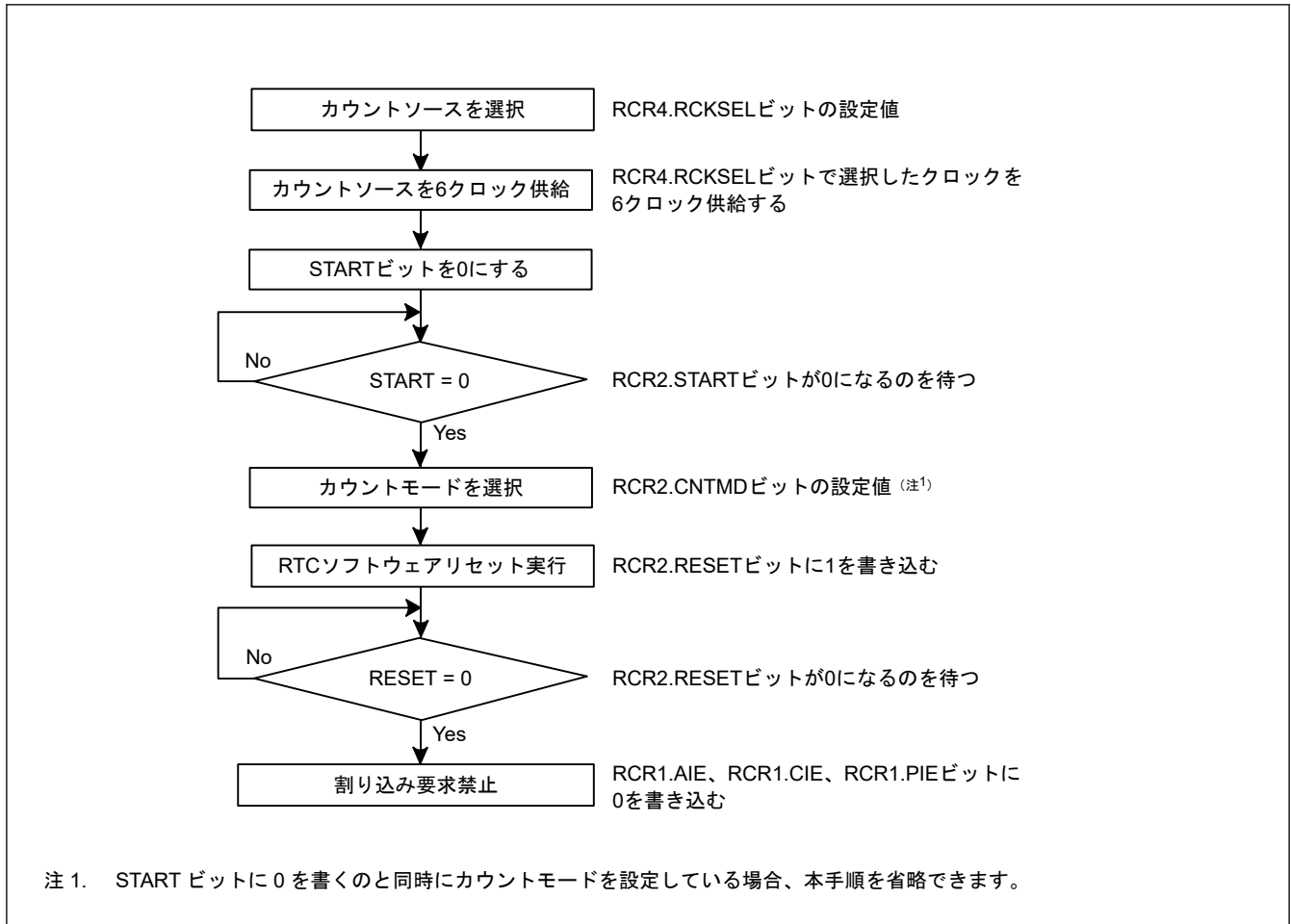
図 22.14 RTC を使用しない場合の初期化手順
