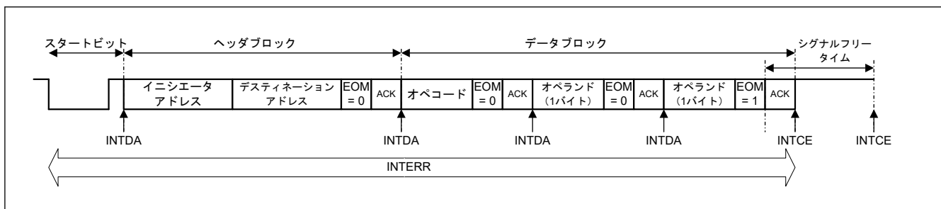
図 31.17 割り込みの発生タイミング
