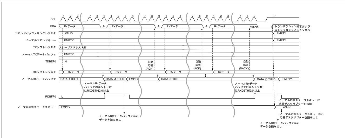
図 27.23 レガシー I3C メッセージデータ読み出し転送タイミング (2/2)
