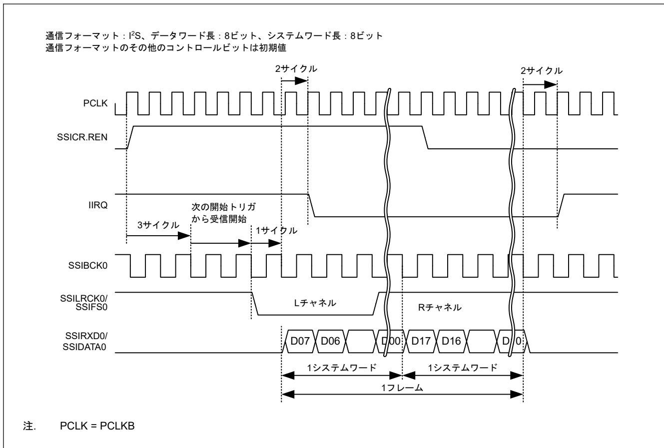
図 32.15 IIRQ 設定タイミング (受信)
