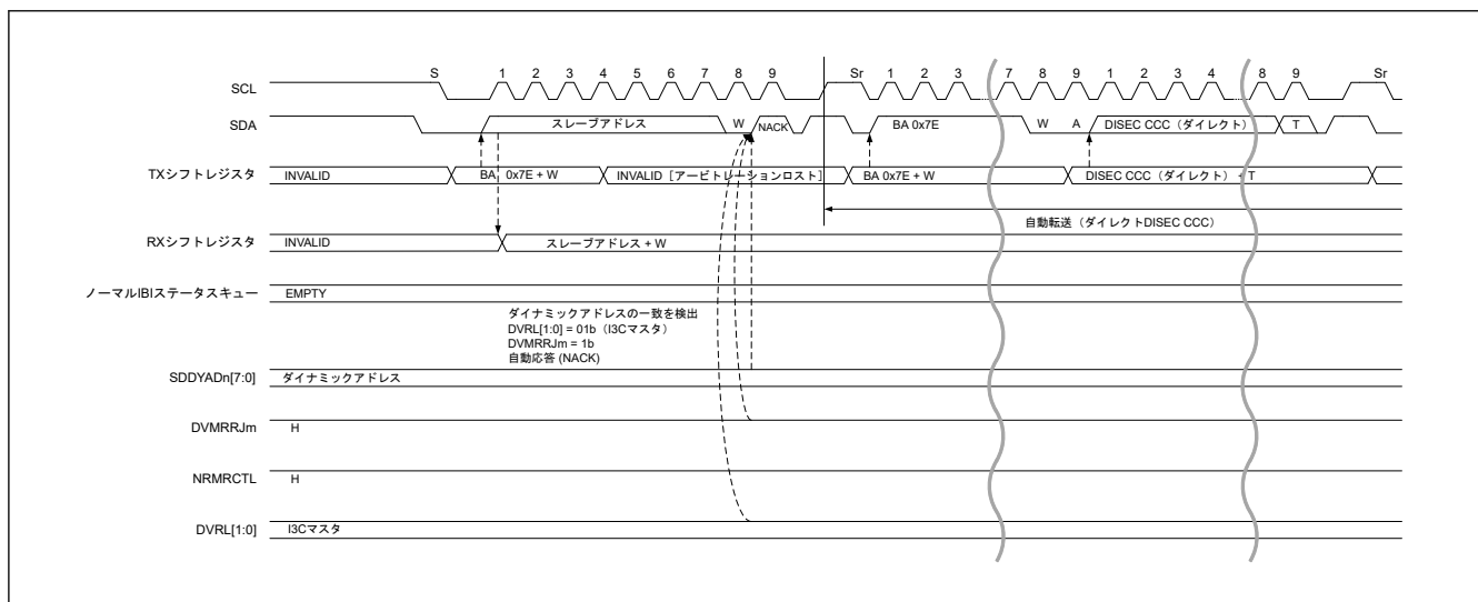
図 27.85 バス権要求 : NACK (DVMRRJ が 1) かつ NRMCTL が 1 の場合 (1/2)
