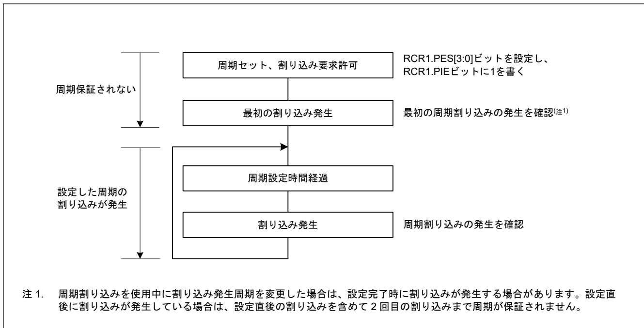
図 22.13 周期割り込み機能の使用法
