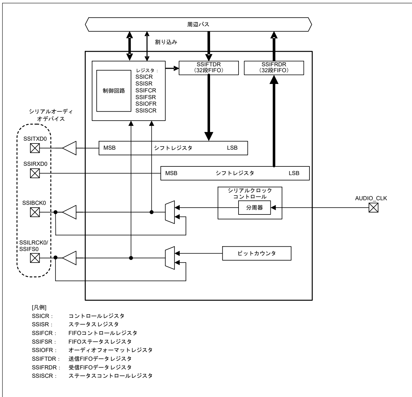
図 32.2 全二重通信の SSIE のブロック図
