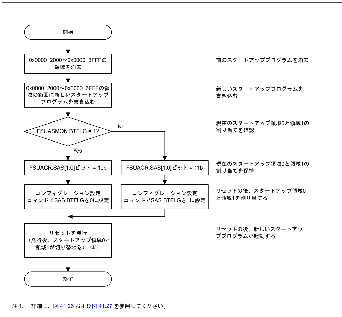
図 41.28 スタートアッププログラム保護の概念
