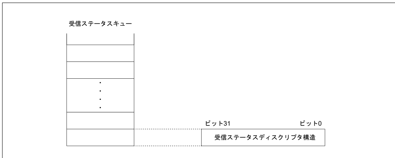
図 27.3 レスポンスディスクリプタデータ構造
