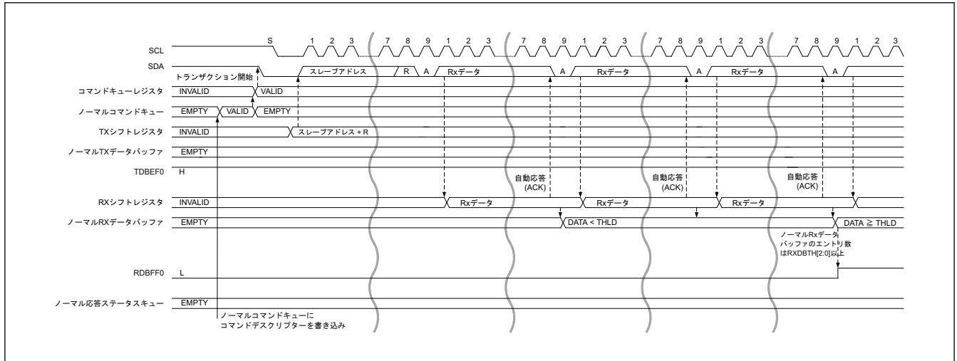
図 27.20 SDR データ読み出し転送タイミング (1/2)
