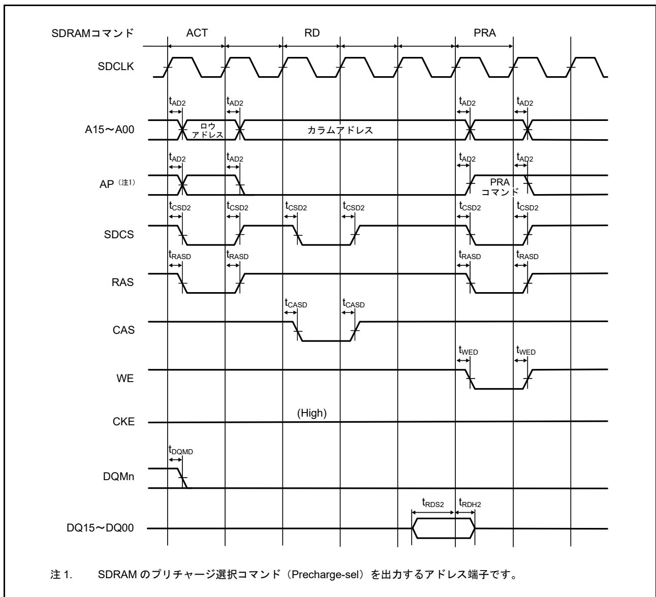
図 60.27 SDRAM シングルリードタイミング
