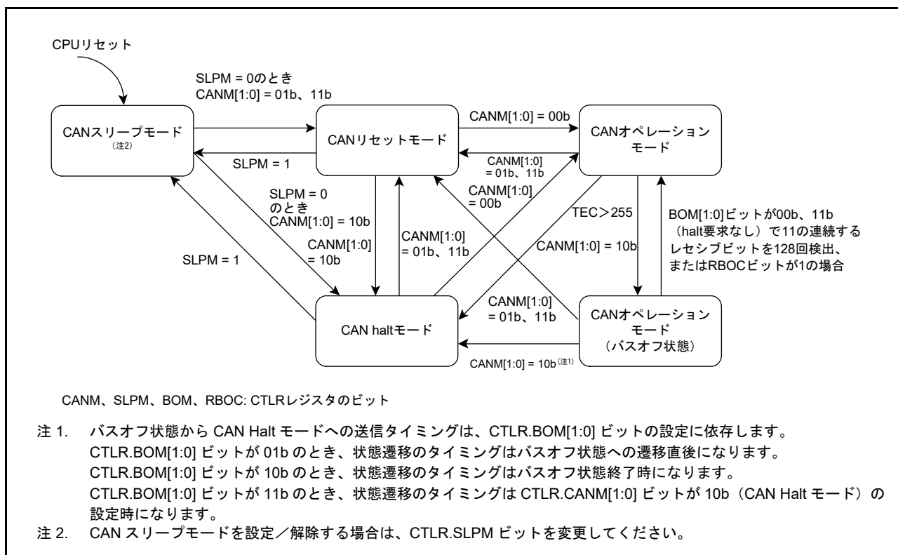
図 37.9 各動作モード間の遷移
