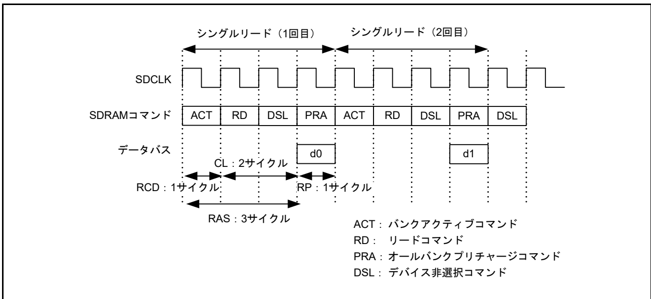
図 15.58 シングルリードタイミング例 (5) (1 転送要求に対して 2 回バスアクセスが発生する場合)
