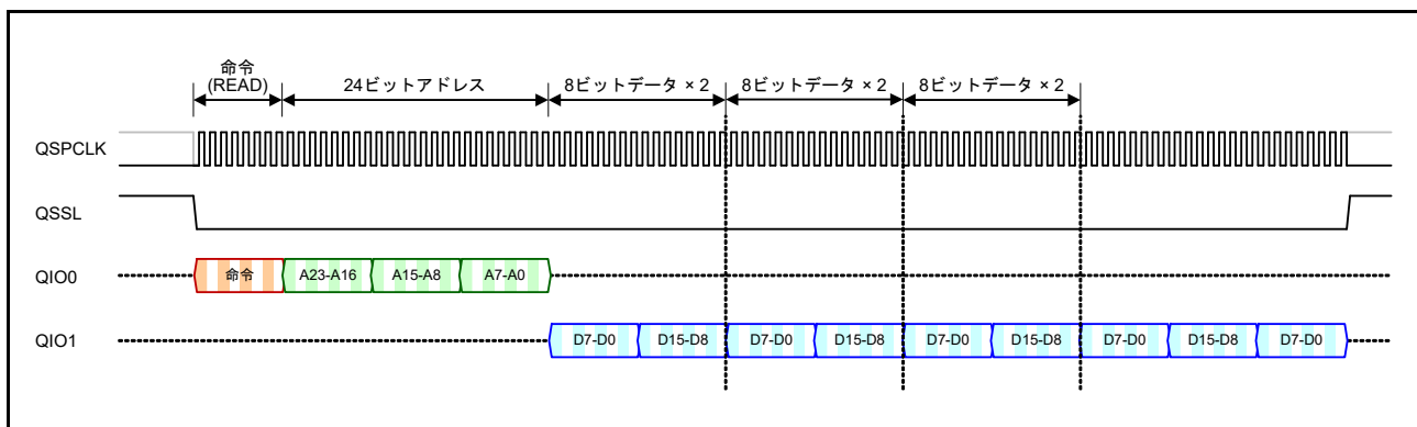
図 39.30 プリフェッチ機能を使用した連続データのリード動作
