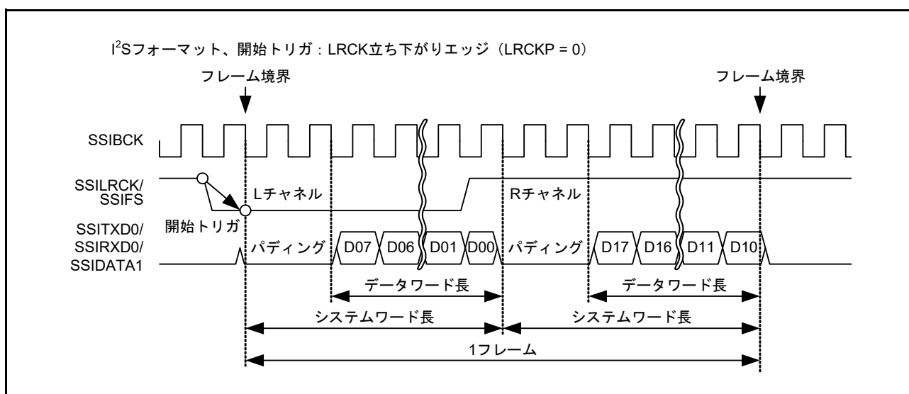
図 41.1 通信フォーマットの定義
