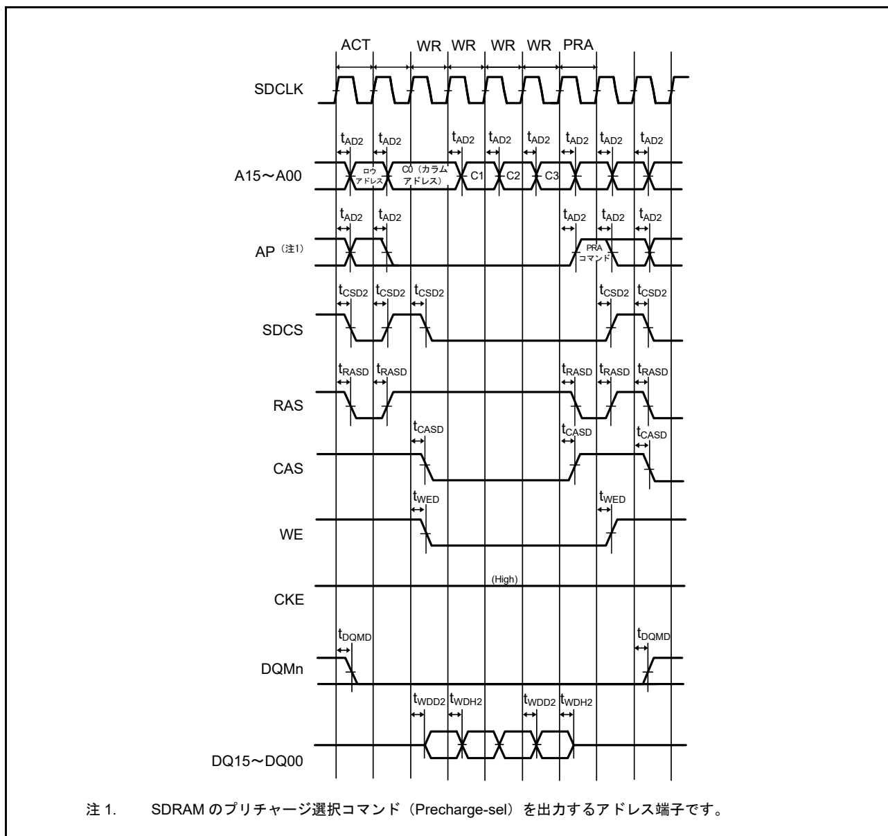
図 60.30 SDRAM 複数ライトタイミング
