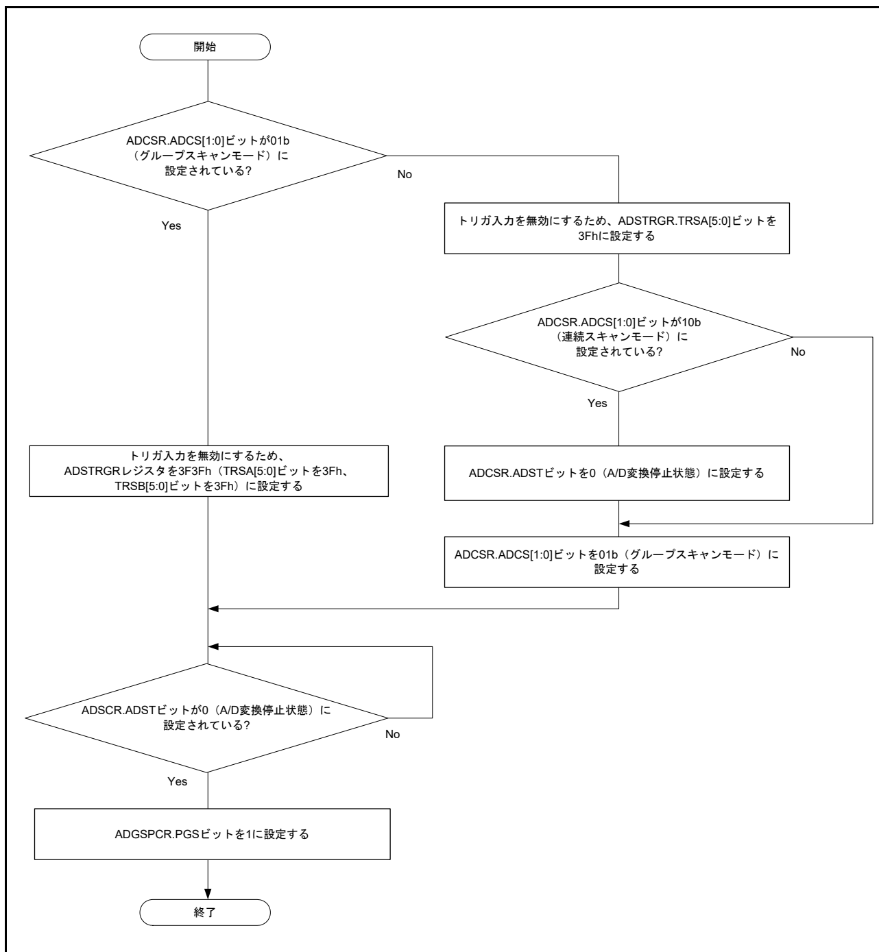
図 47.25 ADGSPCR.PGS ビット 設定時のフロー
