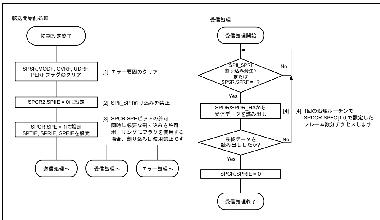
図 38.42 スレーブモードでの受信フロー
