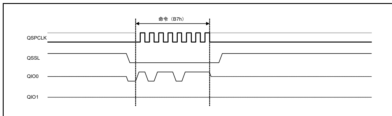
図 39.26 4バイトモード遷移バスサイクル
