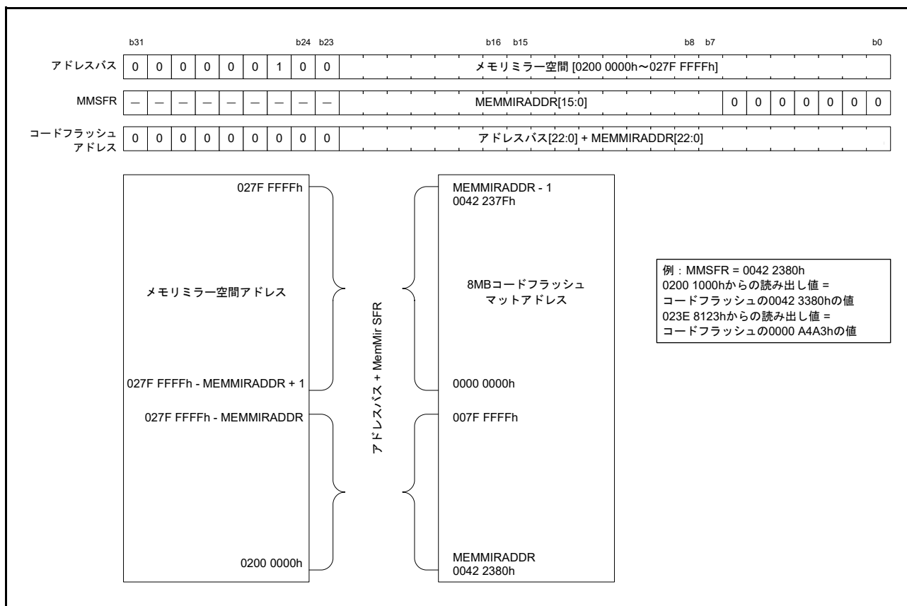
図 5.1 MMF 動作
