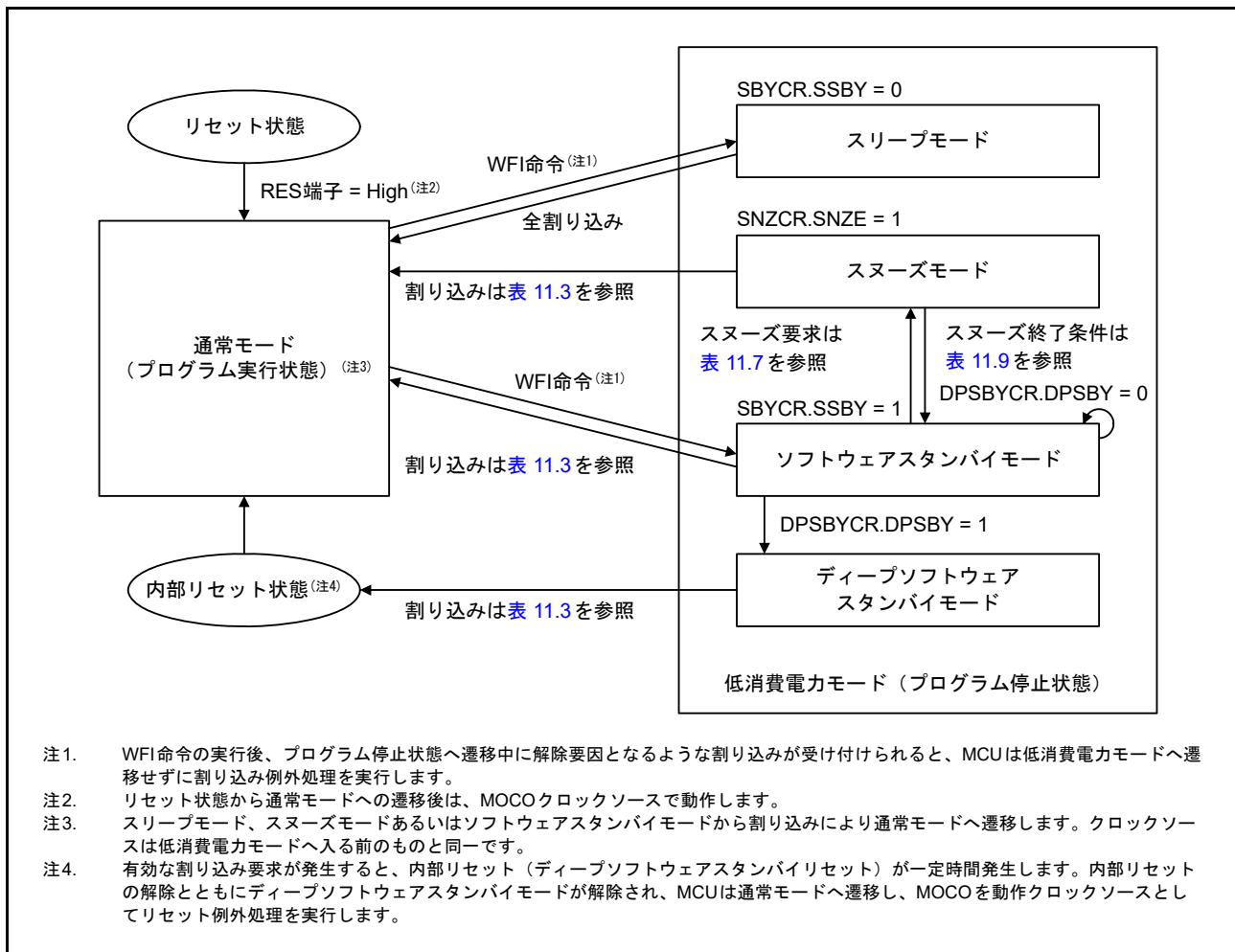
図 11.1 モード遷移
