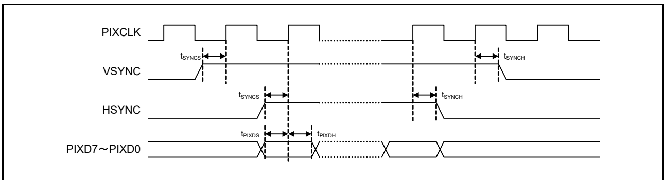
図 60.79 PDC AC タイミング
