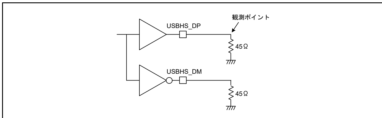
図 60.90 ハイスピードモードにおける測定回路
