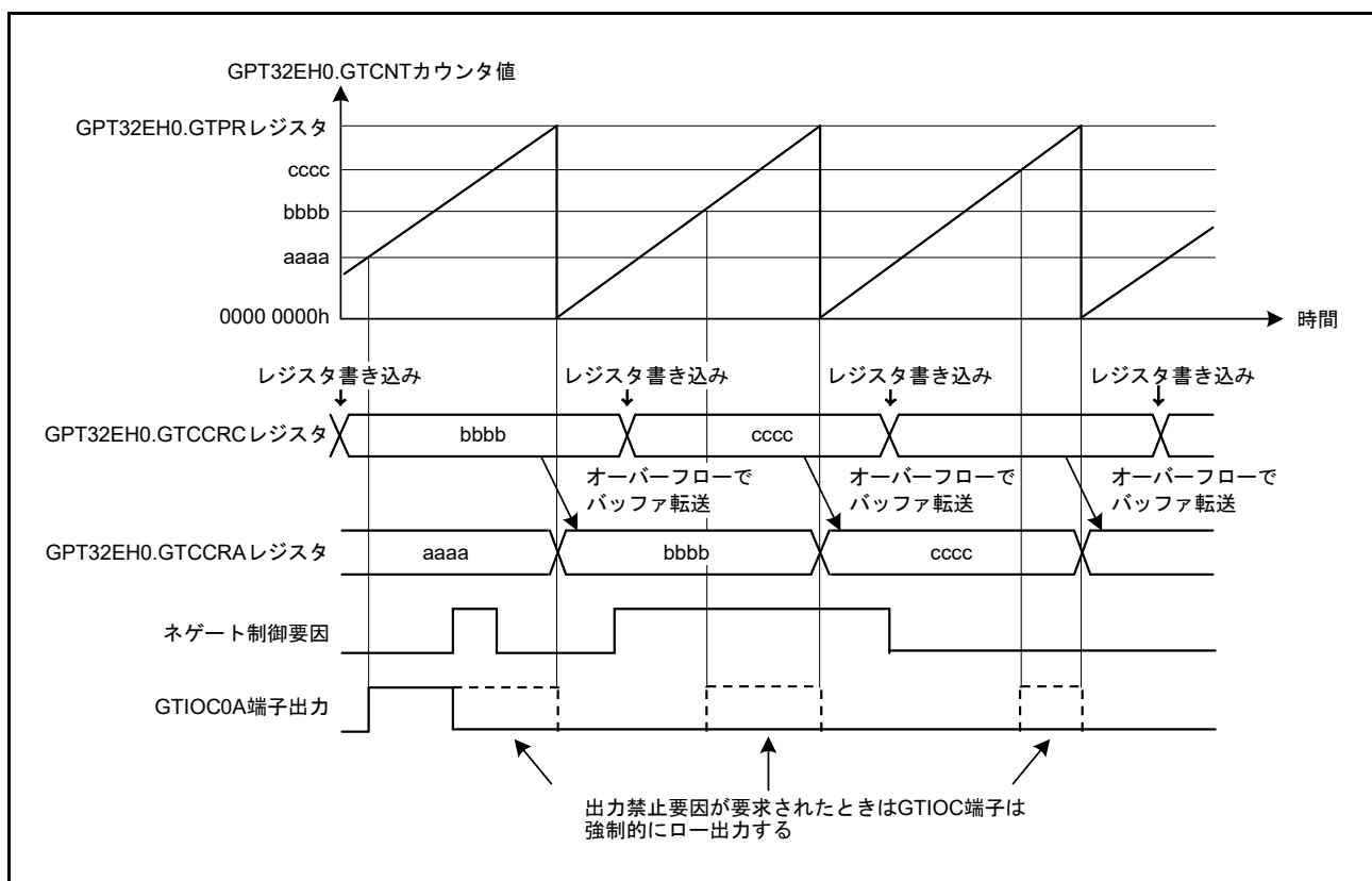
図 23.96 GTIOC 端子出力禁止制御動作例 (のこぎり波でアップカウント、バッファ動作、アクティブレベル1、GTCRA レジスタのコンペアマッチで High 出力、周期の終わりで Low 出力、出力禁止で Low 出力の場合)
