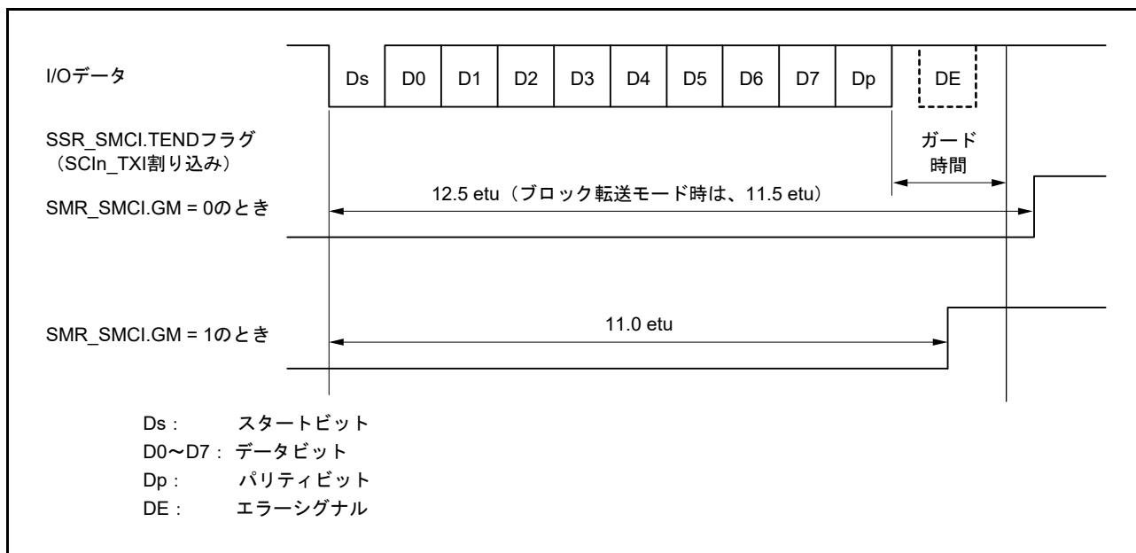
図 34.53 送信中の SSR.TEND フラグの発生タイミング
