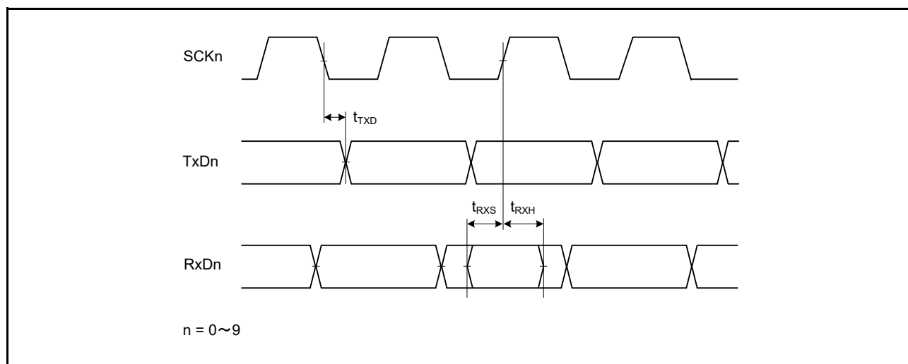
図 60.44 クロック同期式モードにおける SCI 入出力タイミング
