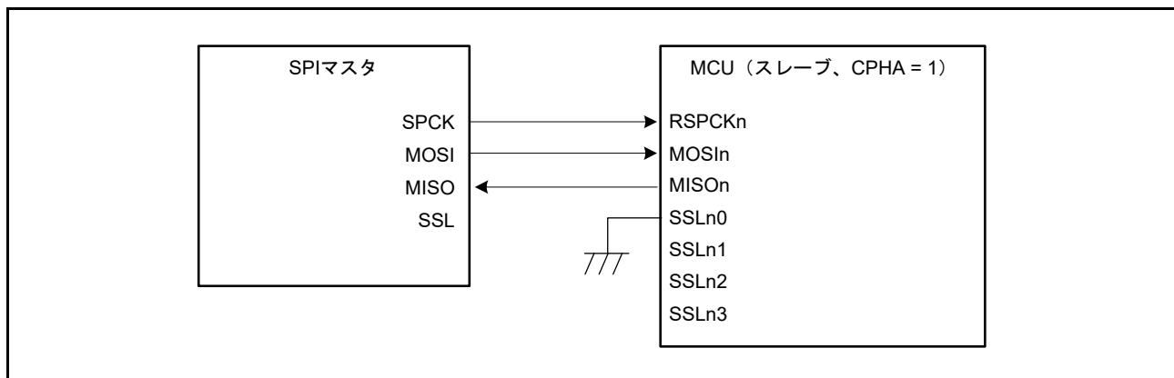
図 38.7 シングルマスタおよびシングルスレーブの構成例 (MCU はスレーブ、CPHA = 1)
