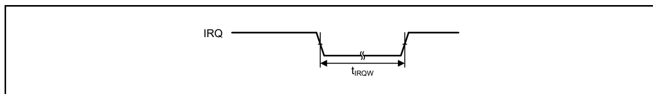
図 60.19 IRQ 割り込み入カタイミング
