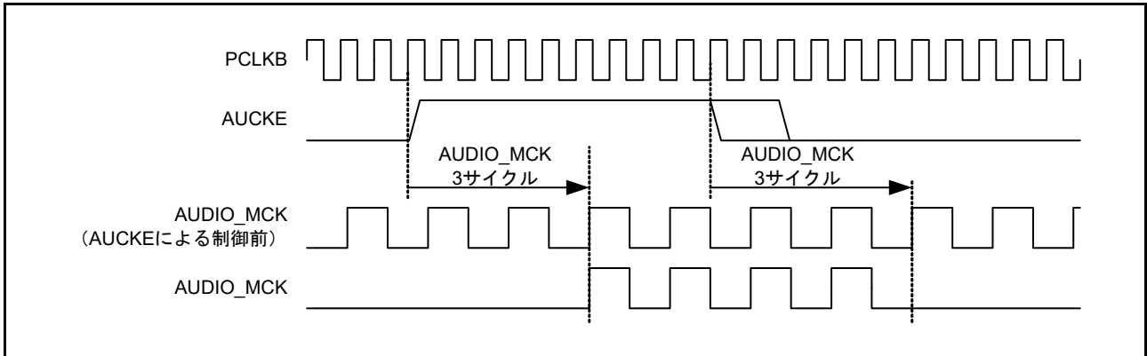
図 41.25 AUDIO_MCK の停止/再開
