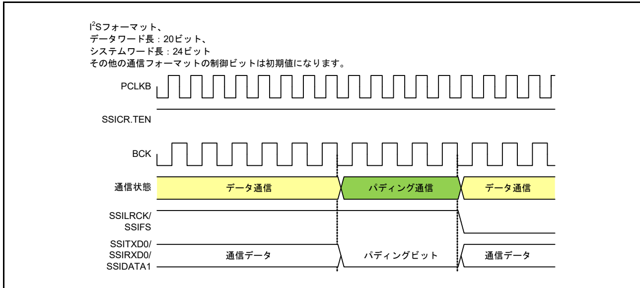
図 41.49 データ通信からパディング通信への遷移
