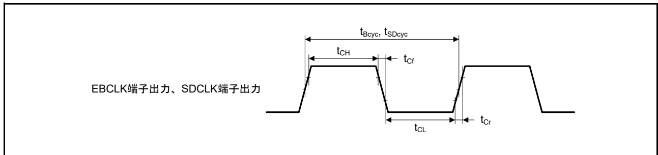
図 60.7 EBCLK および SDCLK の出力タイミング
