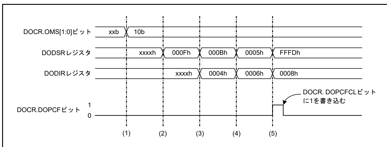
図 52.4 データ減算モードの動作例
