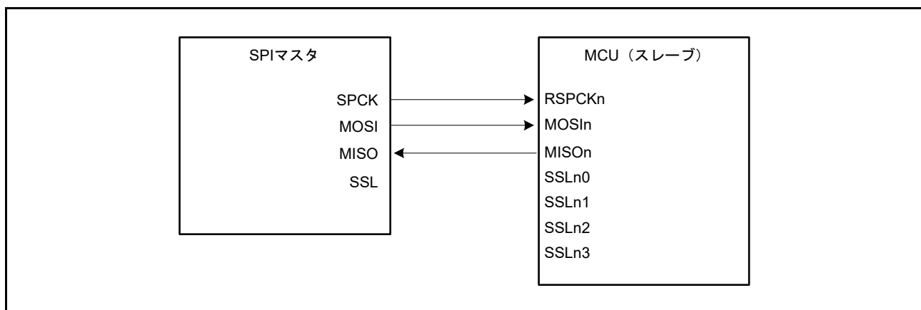
図 38.12 クロック同期式モードでのマスタ/スレーブの構成例 (MCU = スレーブ、CPHA = 1)
