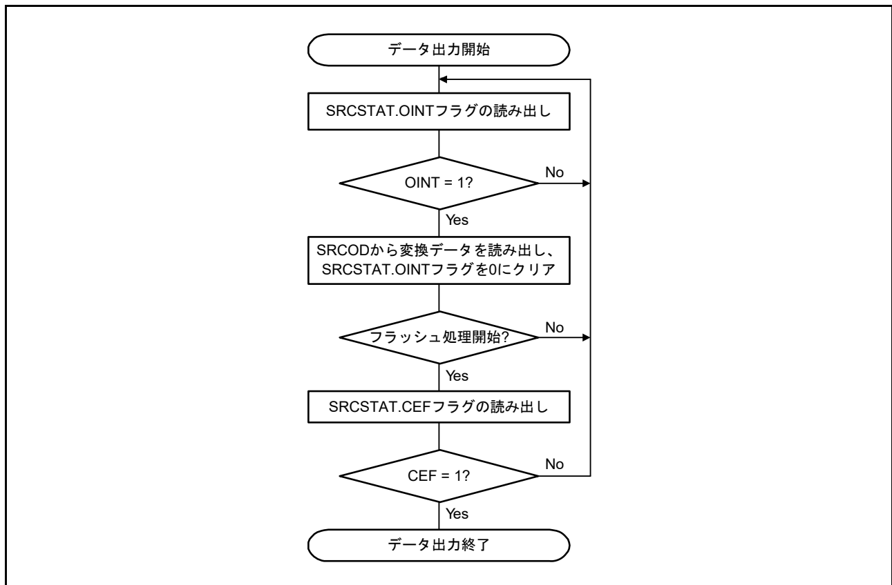
図 42.4 データ出力フロー
