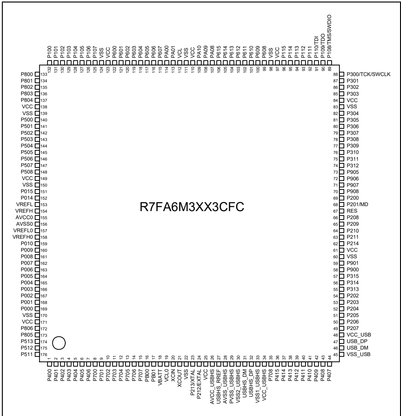
図 1.4 176-pin LQFP のピン配置図 (上面図)
