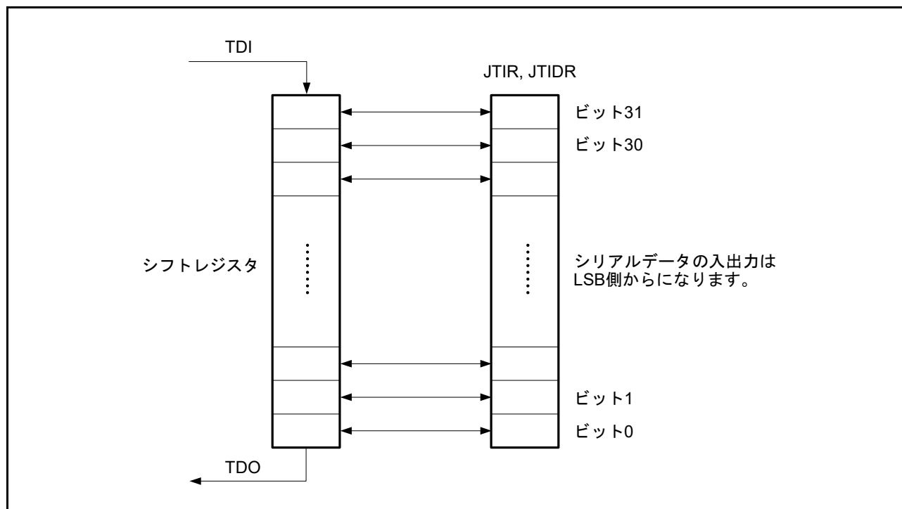
図 45.3 シリアルデータ入出力
