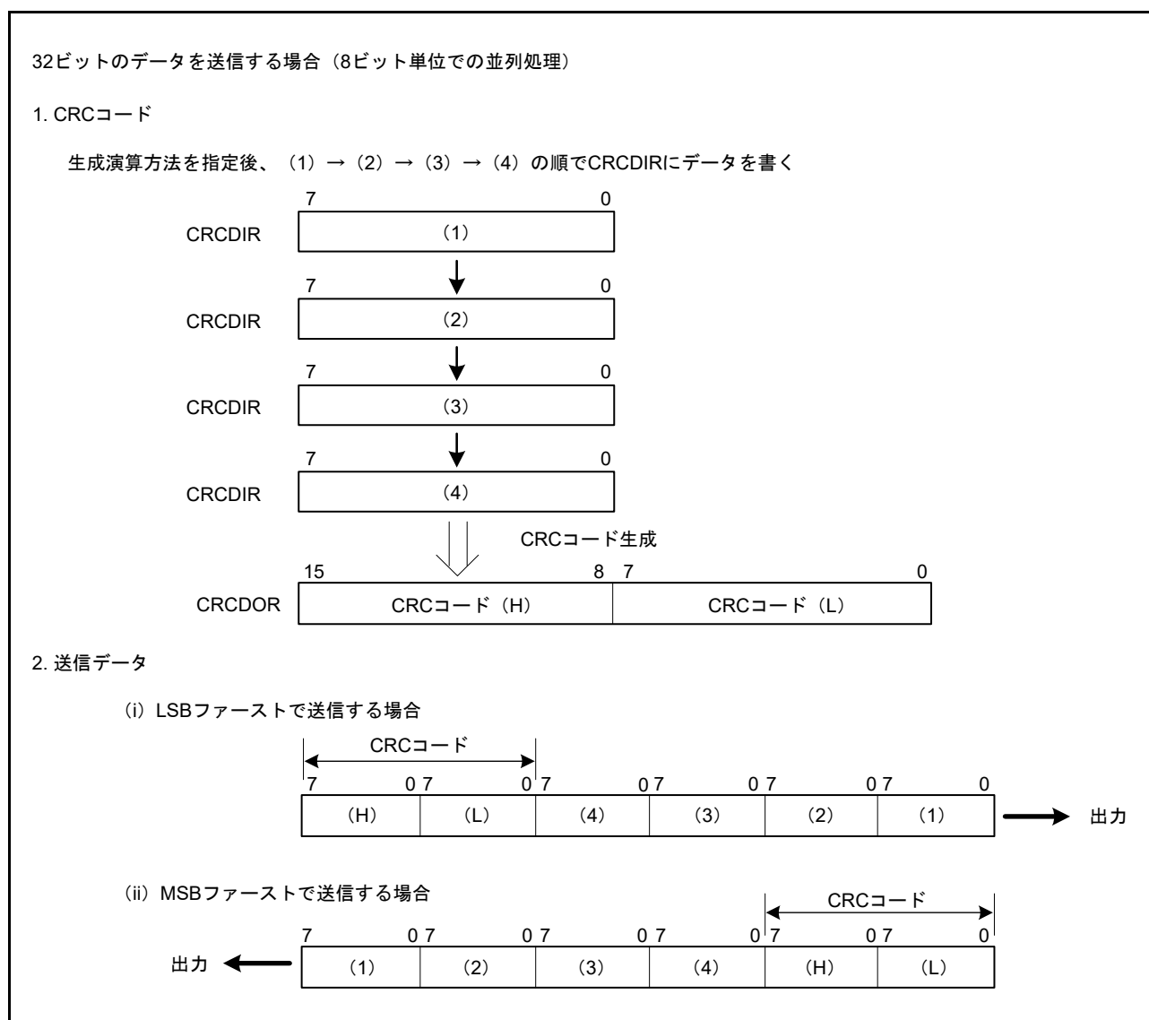
図 40.6 LSB ファーストと MSB ファーストのデータ送信
