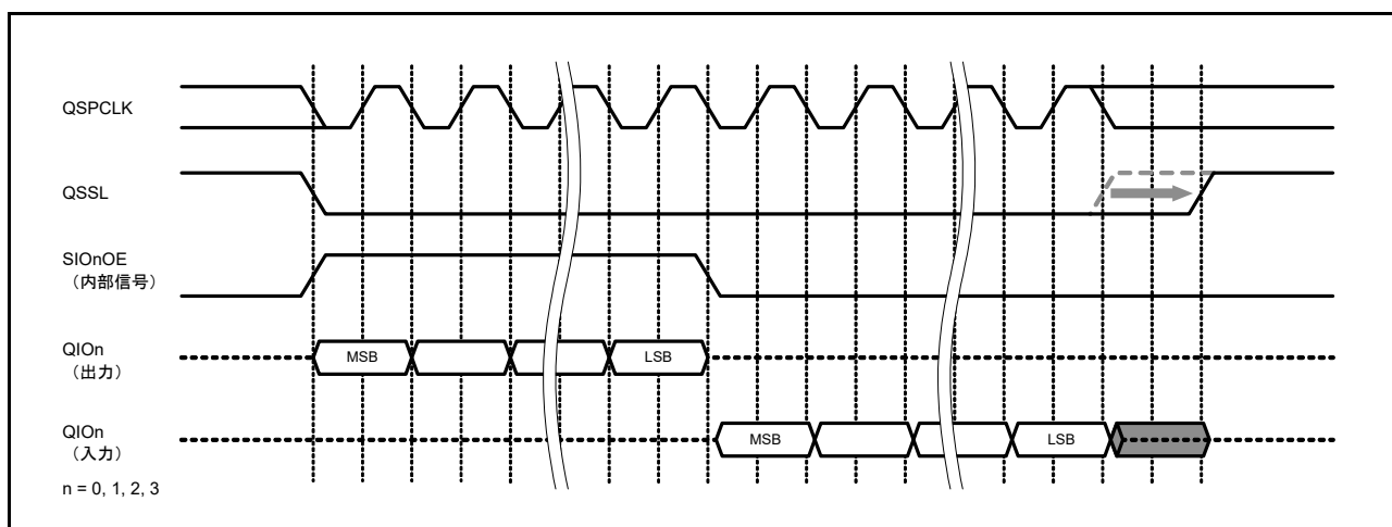
図 39.11 SFMSHD ビットを使用した QSSL 信号のホールド時間調整
