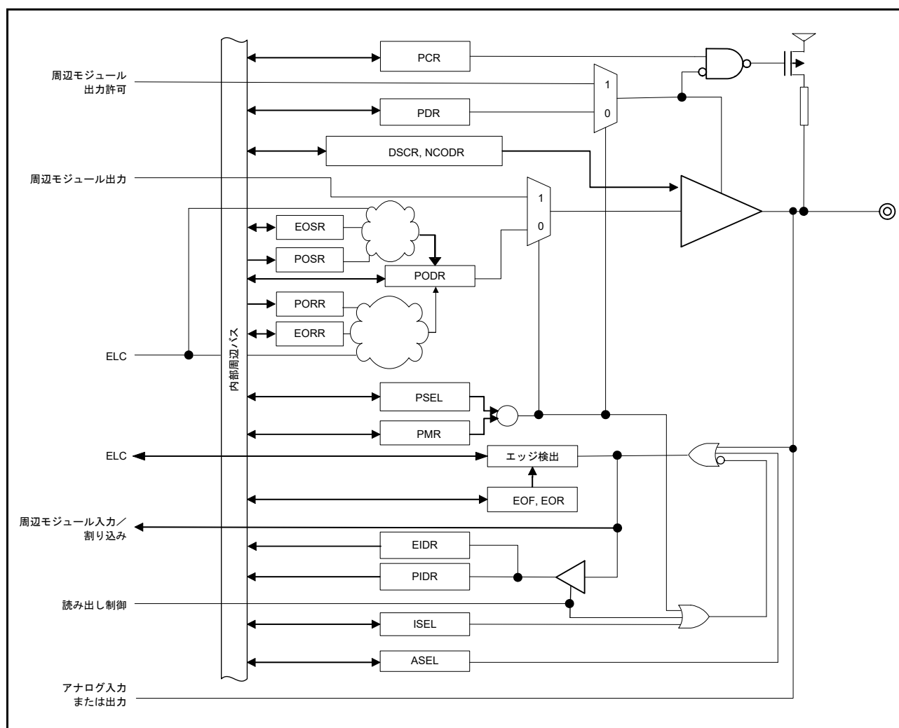
図 20.1 I/Oポートレジスタの接続図
