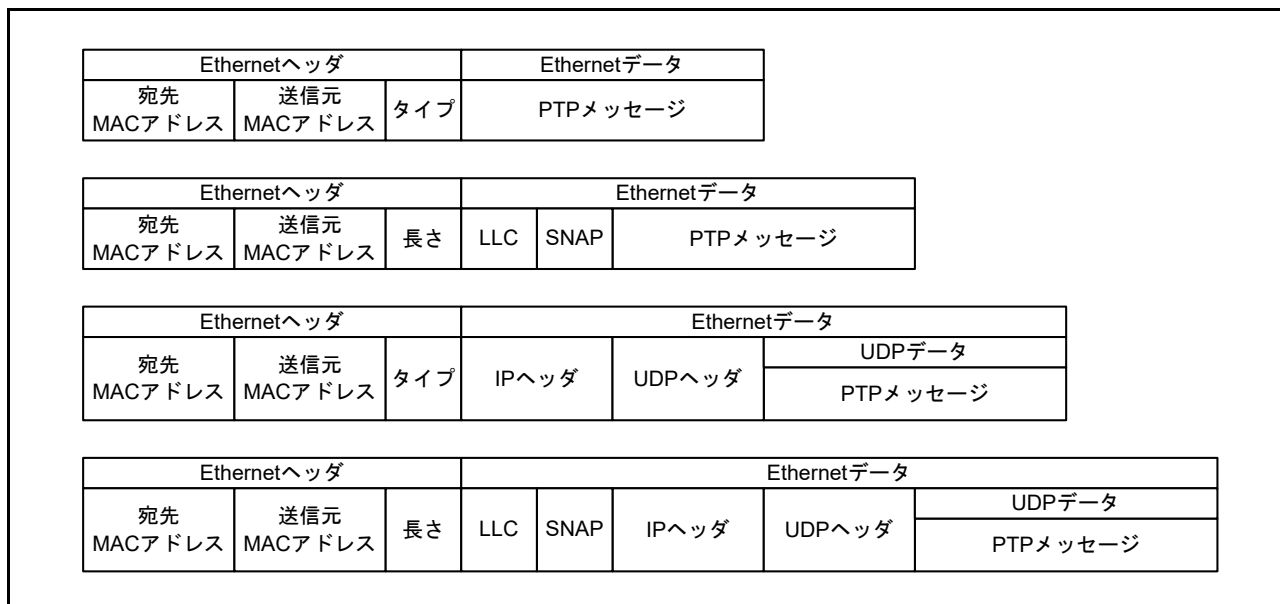
図 30.2 PTPメッセージのフレームフォーマット
