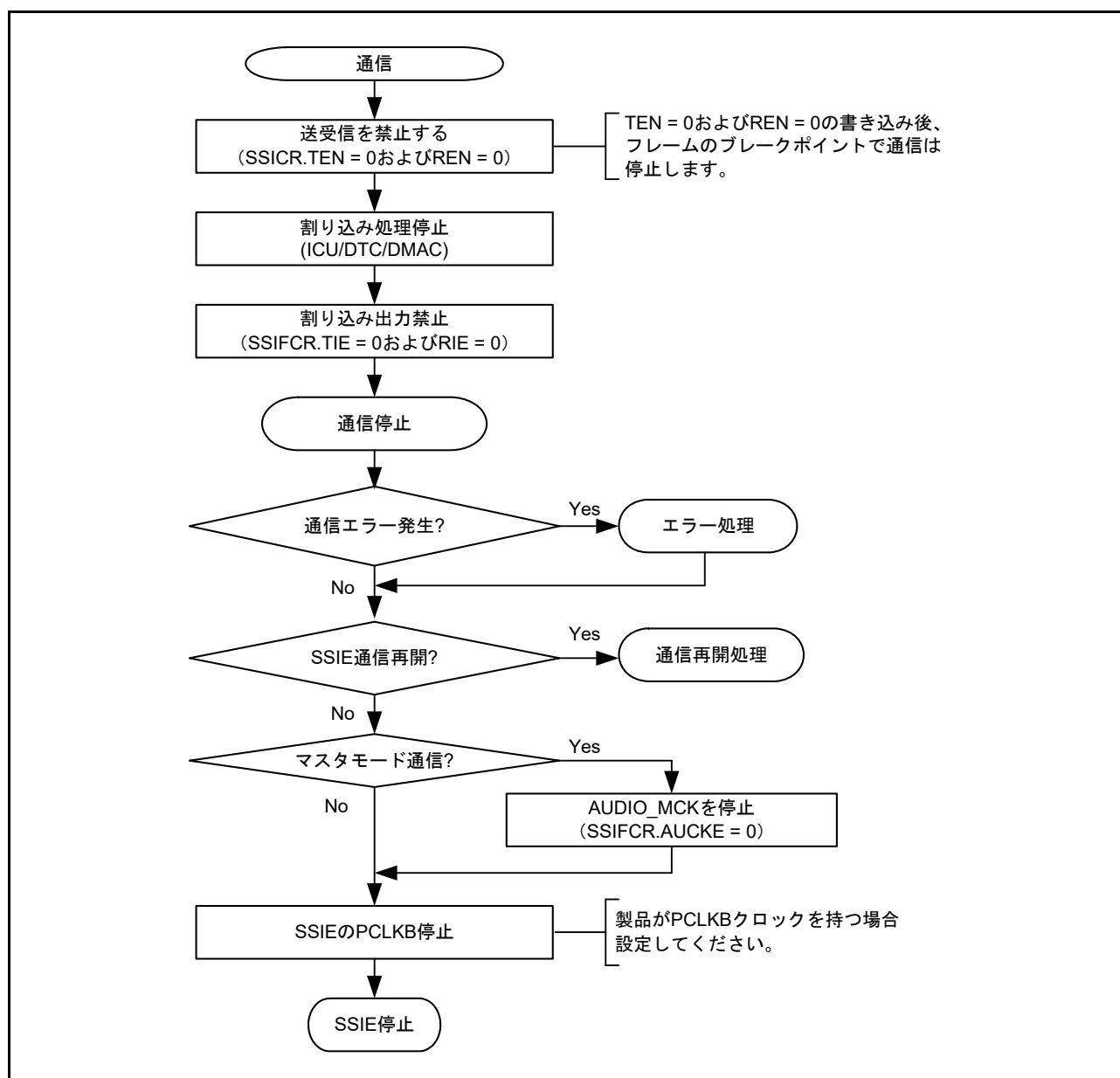
図 41.56 通信停止手順 (CPU 動作手順)
