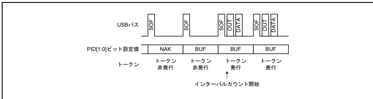
図 33.12 IITV[2:0] = 0 の場合におけるトークン発行の有無
