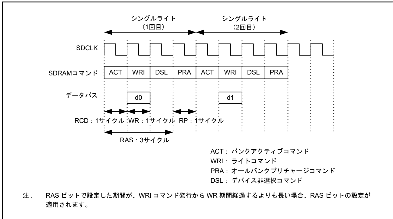
図 15.63 シングルライトタイミング例 (5) (1 転送要求に対して 2 回バスアクセスが発生する場合)
