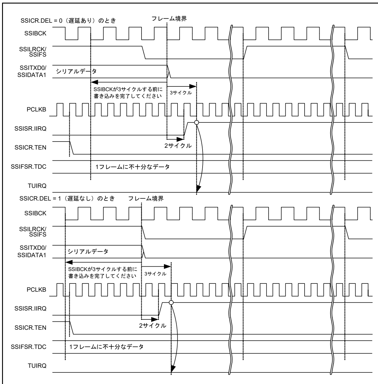
図 41.21 TUIRQ 設定タイミング (通信が停止する場合)
