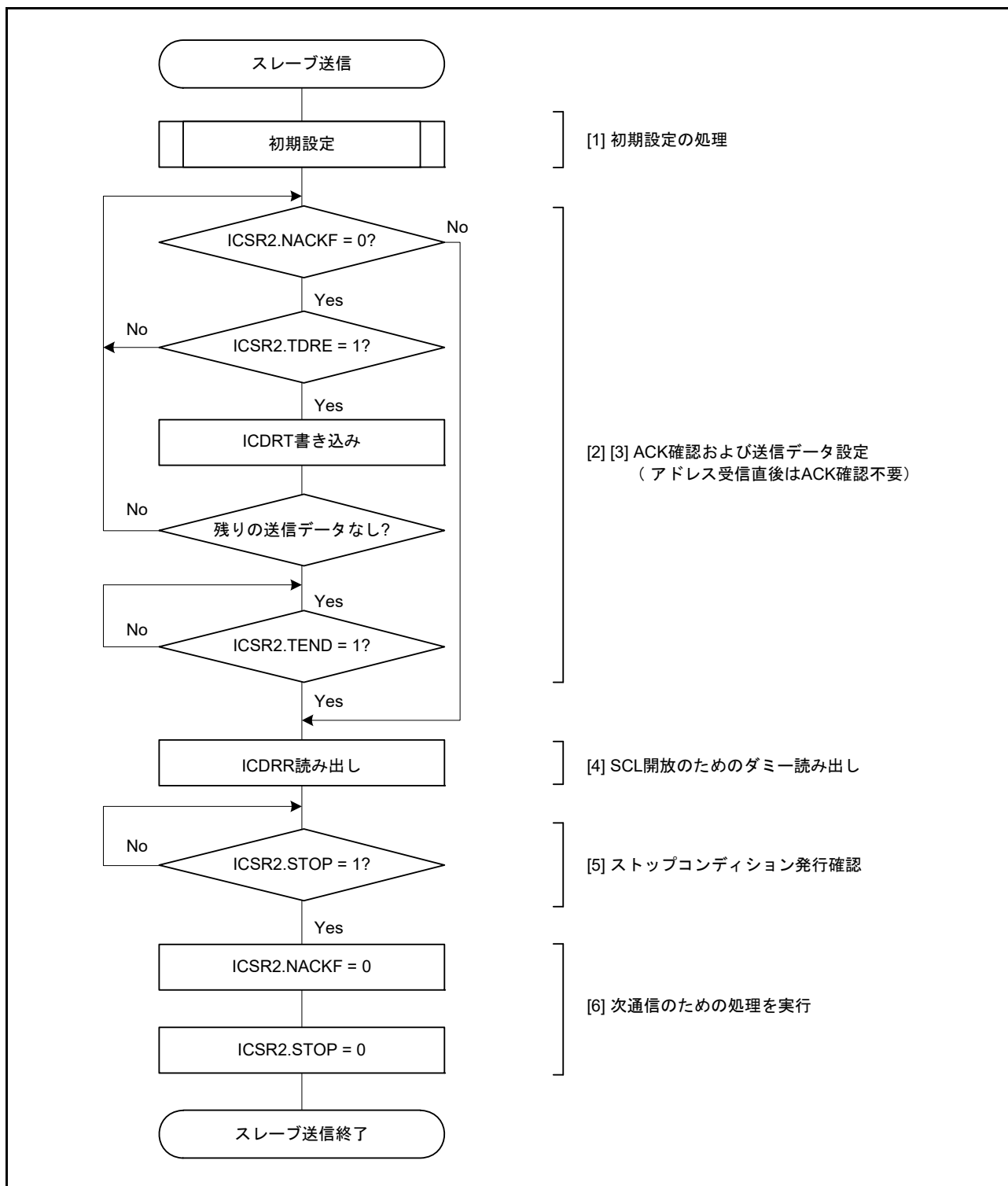
図 36.15 スレーブ送信のフロー例
