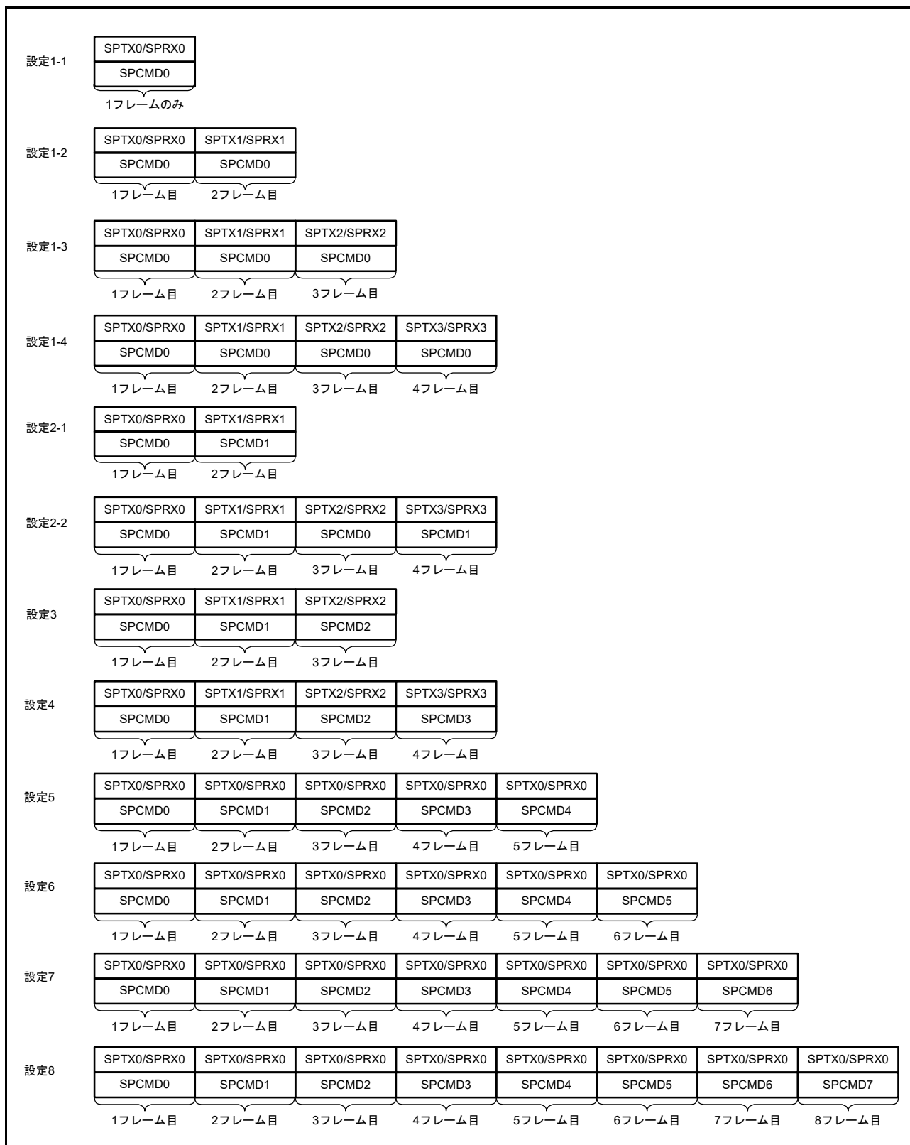
図 38.34 シーケンス動作時の SPI コマンドレジスタと送受信バッファの対応関係
