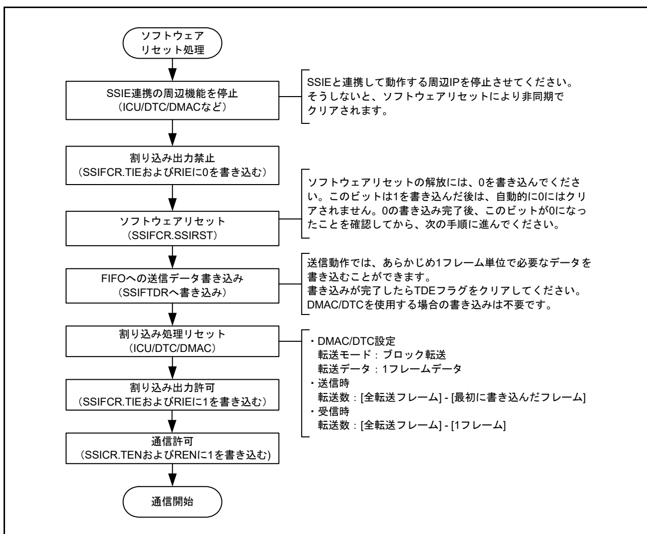
図 41.62 ソフトウェアリセット手順 (CPU 動作手順)
