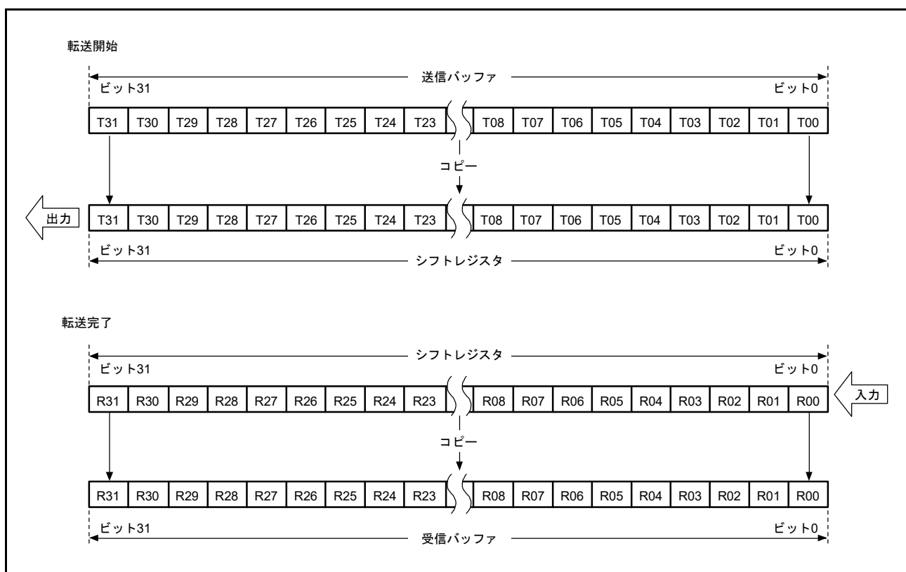
図 38.14 MSB ファースト転送 (32 ビットデータ/パリティ機能無効)
