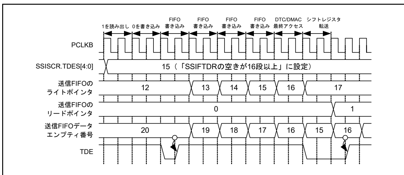
図 41.29 TDE の設定およびクリアのタイミング図
