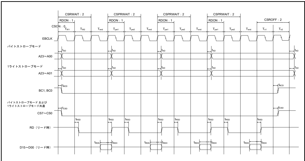
図 60.24 バスクロック同期を使用したページリードサイクルの外部バスタイミング
