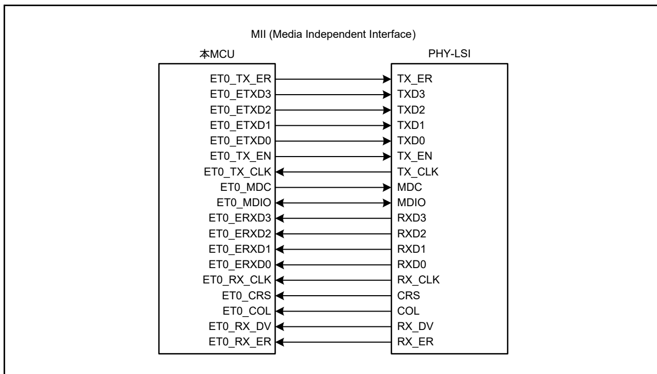
図 29.2 PHY-LSI との接続例 (MII)
