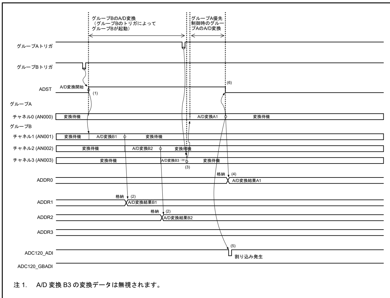
図 47.29 グループ A 優先制御の動作例 (4) (ADGSPCR.GBRSCN = 0、ADGSPCR.GBRP = 0 の場合)
