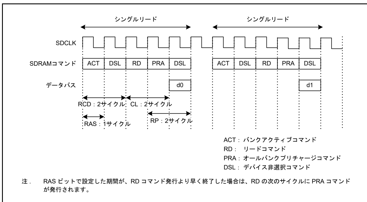
図 15.55 シングルリードタイミング例 (2)
