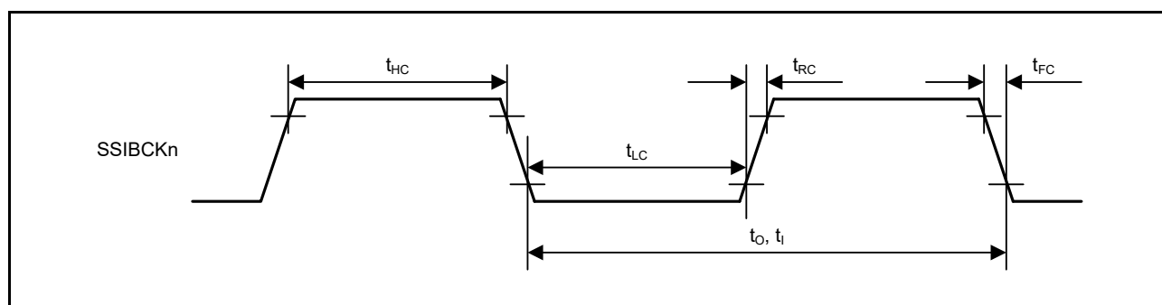
図 60.61 SSIE クロック入出力タイミング
