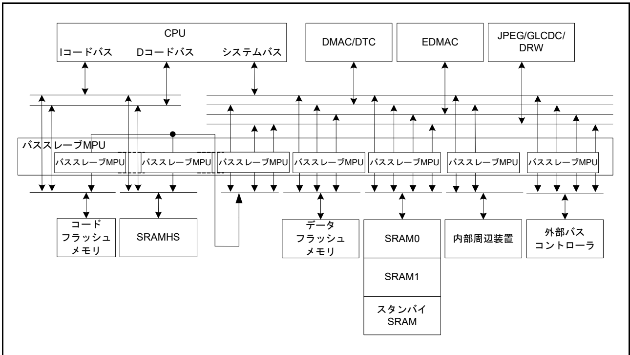
図 16.9 バススレーブ MPU ブロック図
