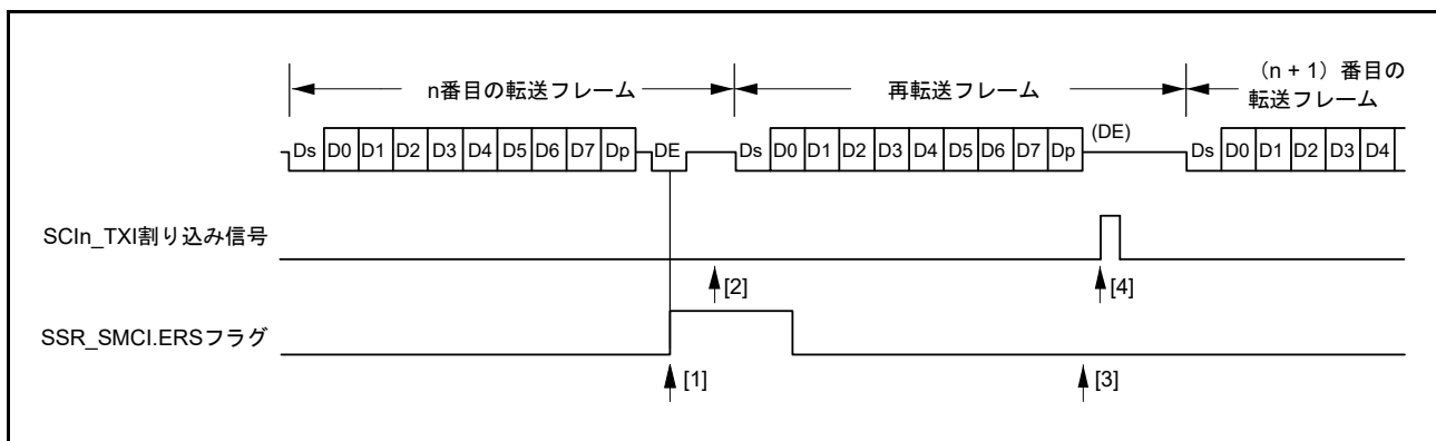
図 34.52 SCI 送信モードでの再転送動作
