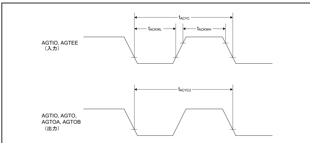
図 60.40 AGT 入出力タイミング
