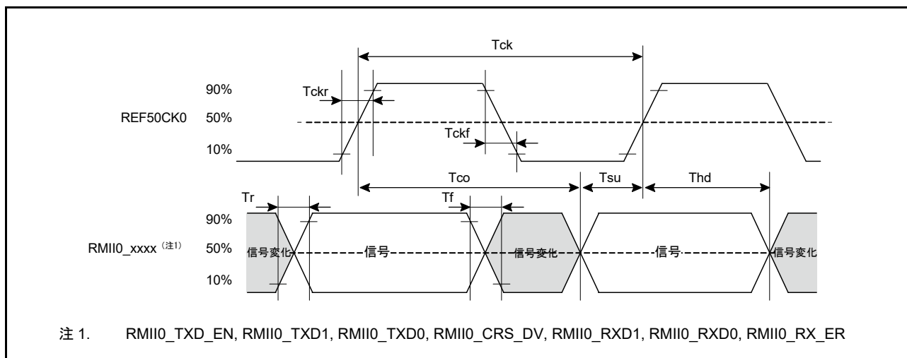
図 60.67 REF50CK0、RMII の信号タイミング
