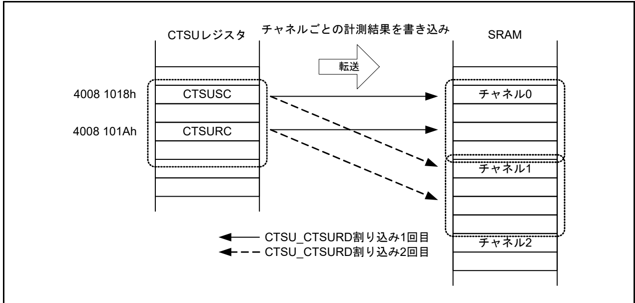
図 51.20 CTSUSURD 割り込みを用いた DTC 転送動作例
