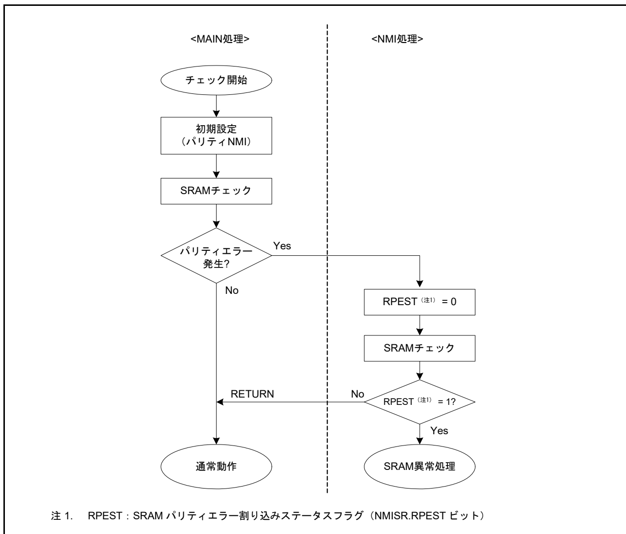
図 53.3 SRAM パリティ割り込み許可の場合の SRAM パリティチェックのフロー
