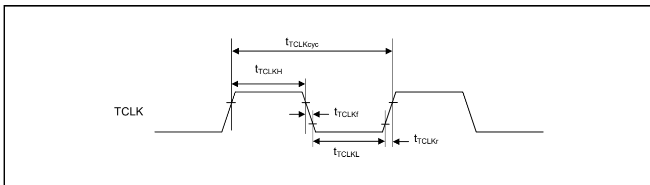
図 60.110 ETM TCLK タイミング
