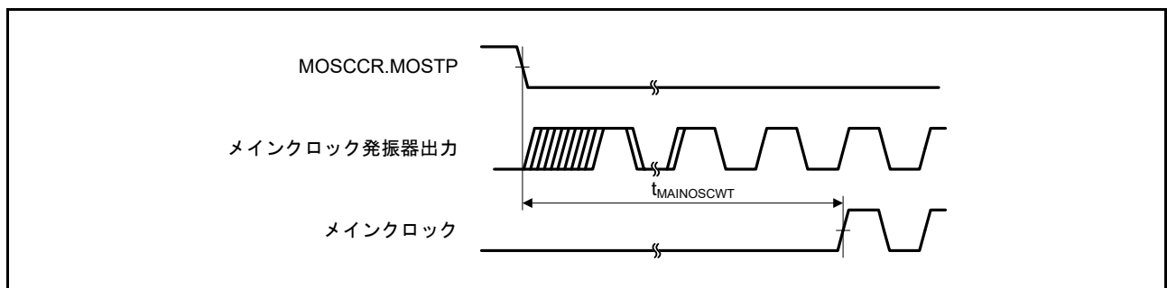
図 60.9 メインクロック発振開始タイミング
