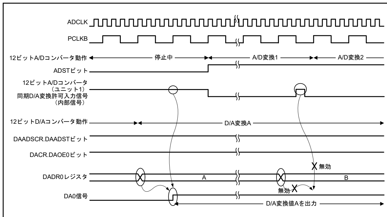
図 48.4 DAC12 が ADC12 (ユニット 1) からの同期 D/A 変換許可入力信号を取り込めない場合の例
