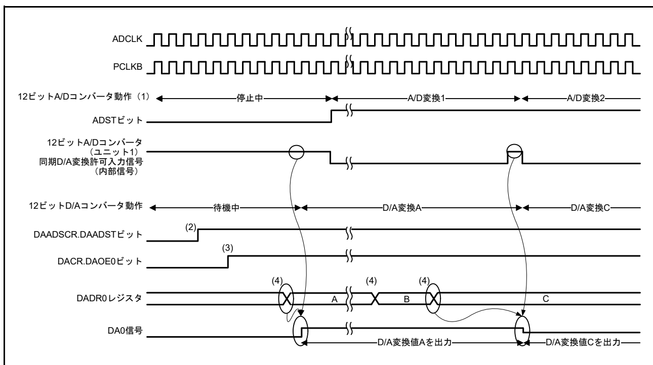
図 48.3 DAC12 を ADC12 に同期して変換する例
