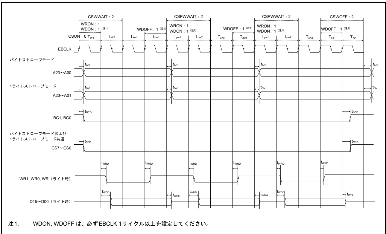
図 60.25 バスクロック同期を使用したページライトサイクルの外部バスタイミング
