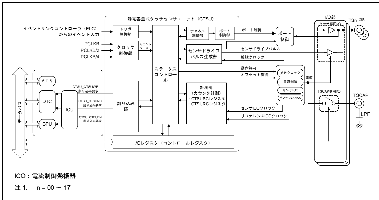
図 51.3 CTSUのブロック図
