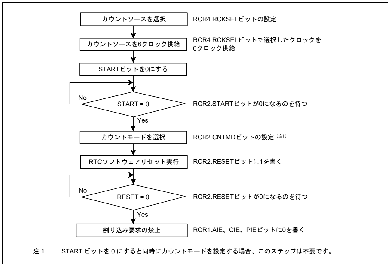
図 26.14 初期化手順
