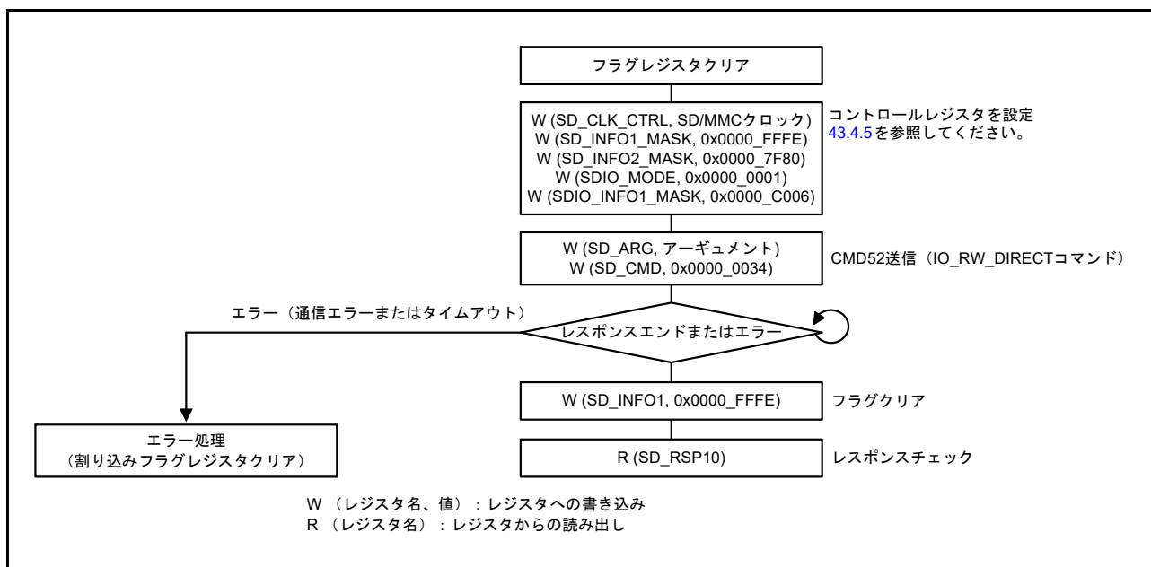
図 43.16 IO_RW_DIRECT コマンド (CMD52) 動作の例
