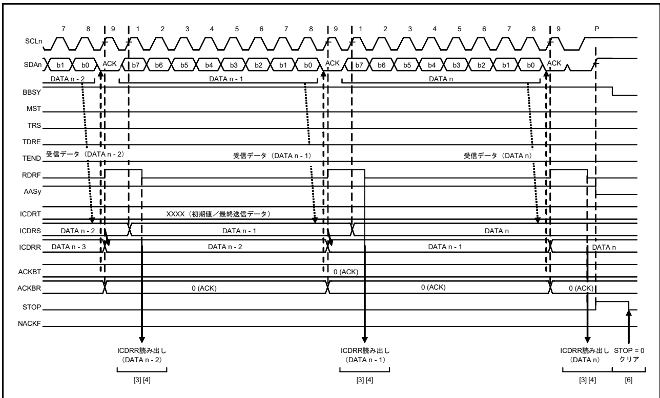
図 36.20 スレーブ受信の動作タイミング (2) (RDRFS = 0 の場合)
