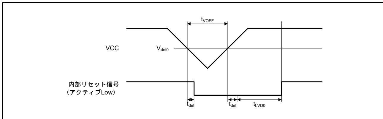
図 60.98 電圧検出回路タイミング ( V_{det0} )
