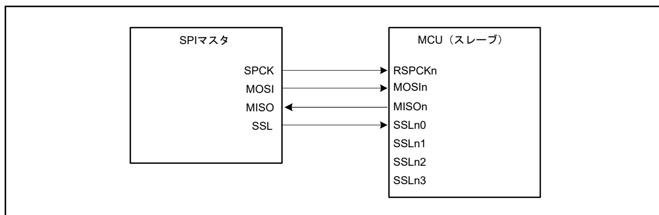
図 38.6 シングルマスタおよびシングルスレーブの構成例 (MCU はスレーブ、CPHA = 0)
