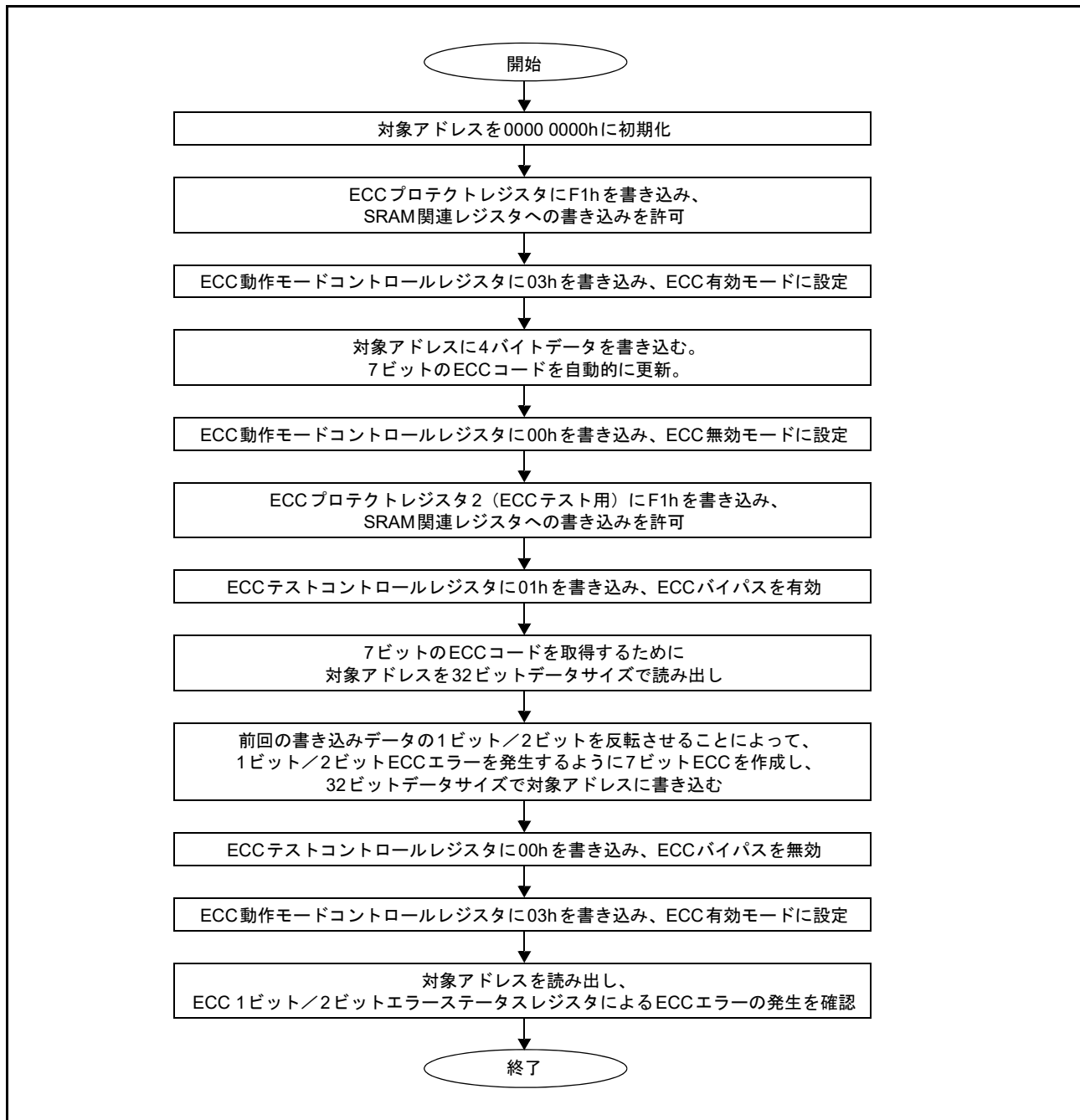
図 53.1 ECC デコーダのテスト方法
