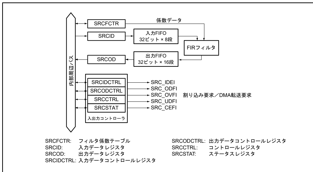
図 42.1 SRCのブロック図
