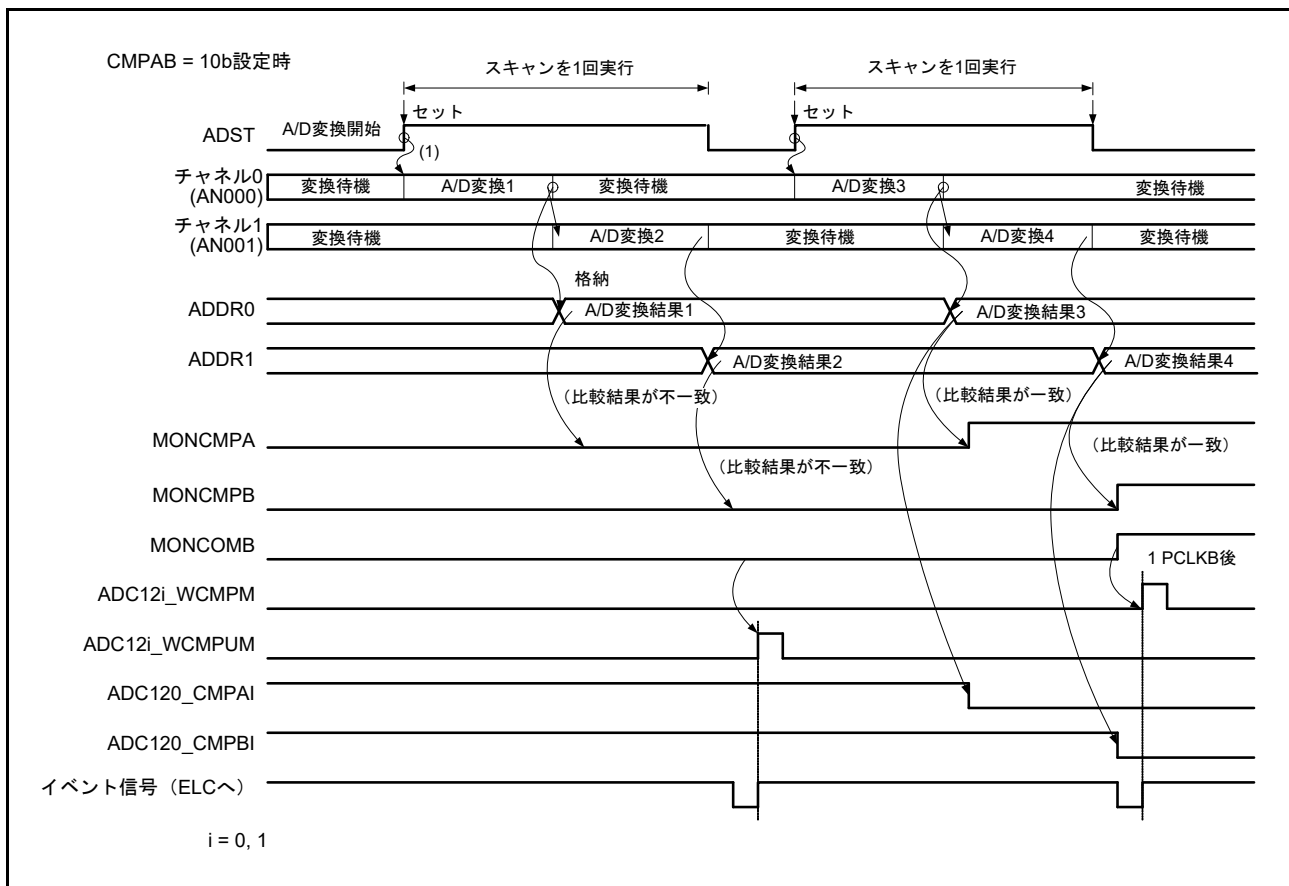
図 47.33 コンペア機能のイベント出力動作例 (AN000 ~ AN001 を比較)
