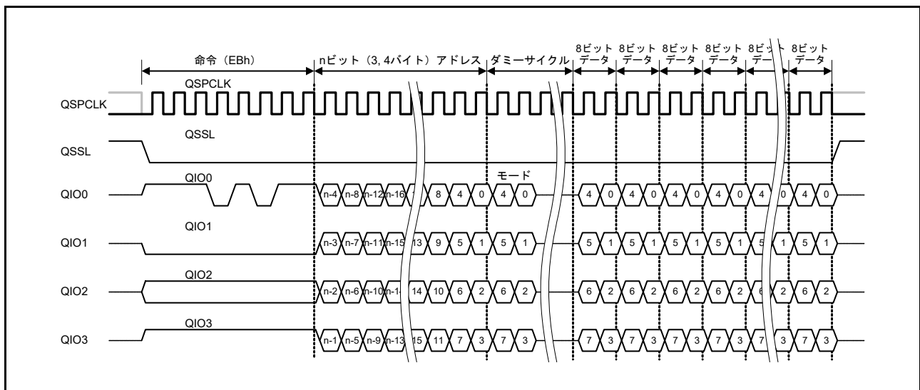
図 39.24 ファストリード Quad I/O バスサイクル
