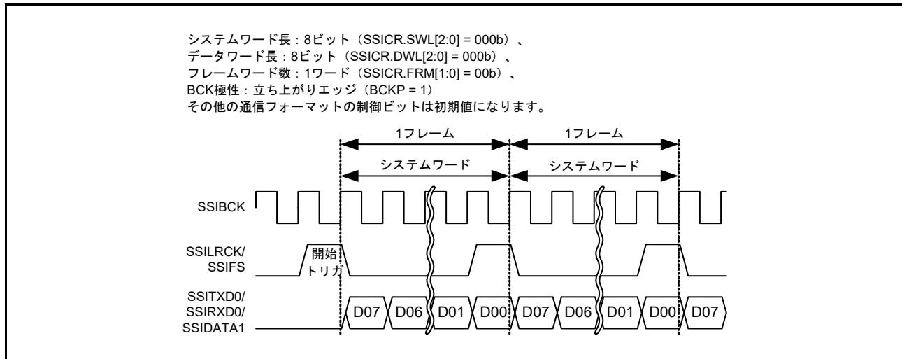
図 41.38 モノラルフォーマットでのショートフレーム (パディングなし、システムワード長 = データワード長)
