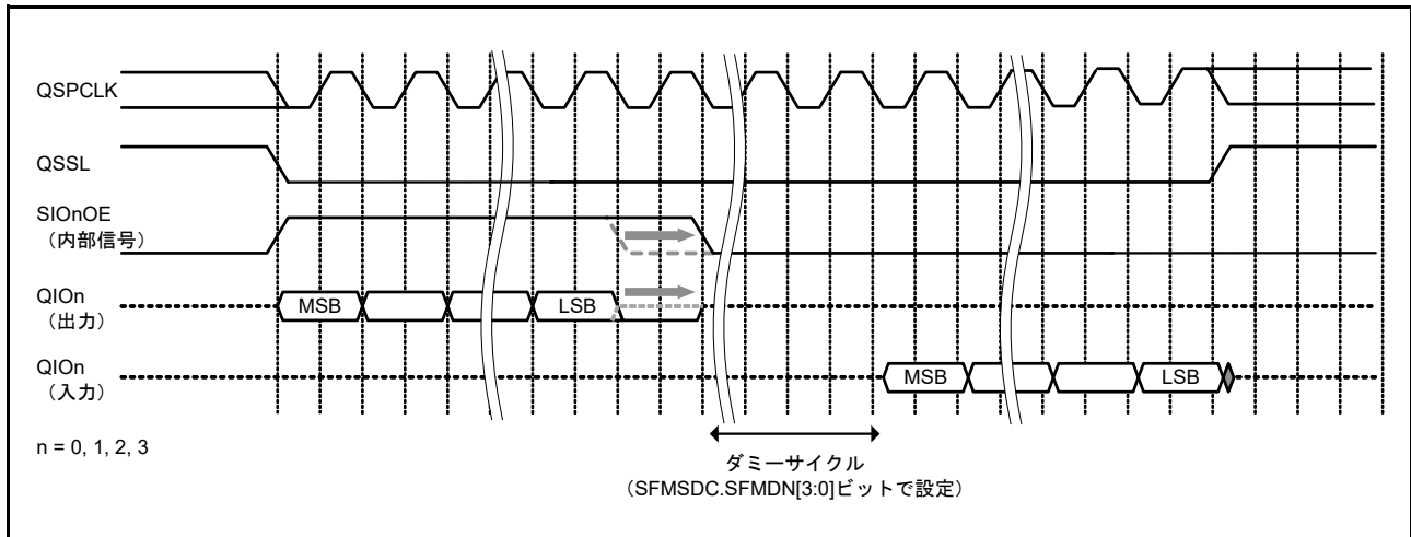
図 39.12 SFMOEX ビットを使用した出力許可ホールド時間調整
