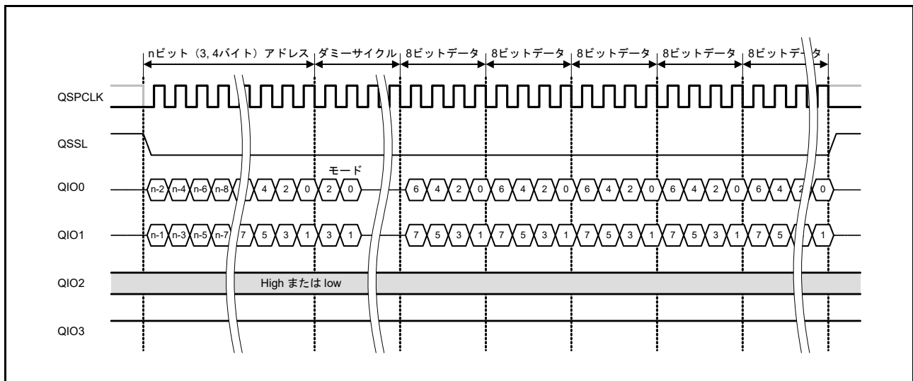
図 39.21 XIP モード時のファストリード Dual I/O バスサイクル
