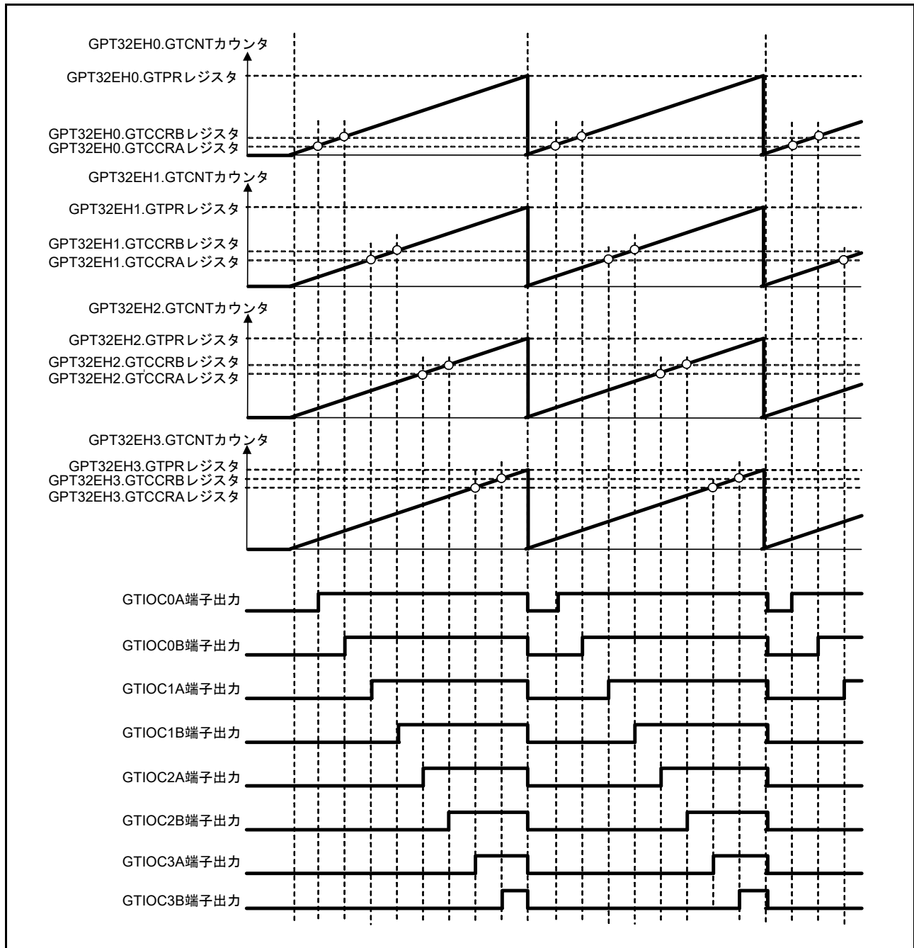
図 23.65 同期 PWM 出力例
