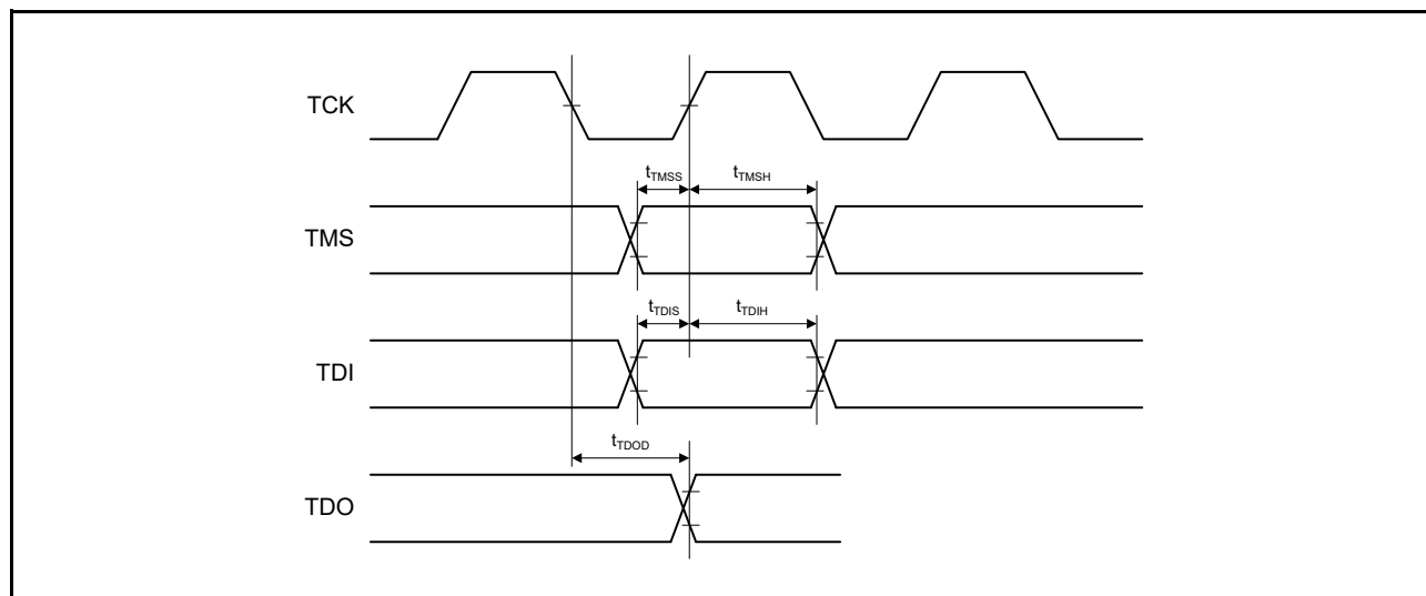
図 60.104 バウンダリスキャン入出力タイミング
