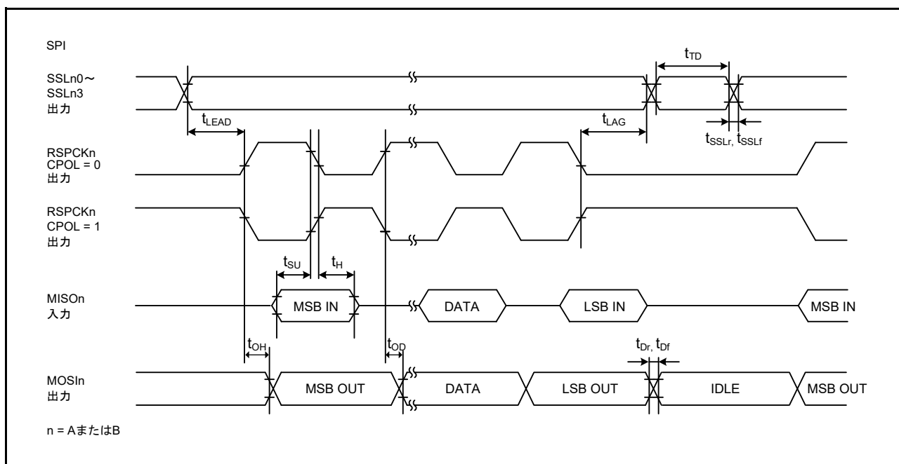
図 60.54 CPHA = 1 の場合におけるマスタの SPI タイミング
