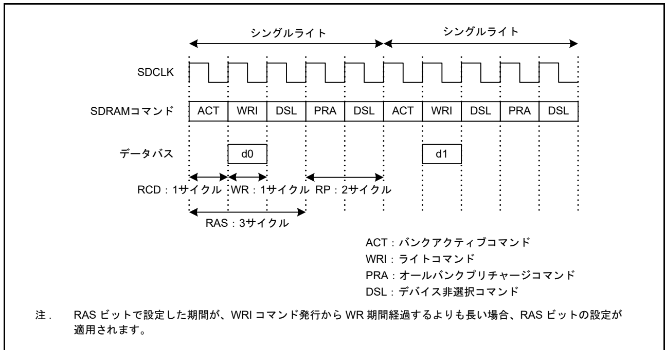
図 15.59 シングルライトタイミング例 (1)
