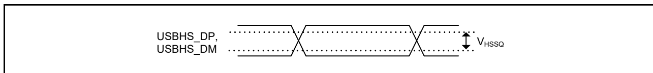
図 60.87 ハイスピードモードにおける USBHS_DP、USBHS_DM の Squelch 検出感度
