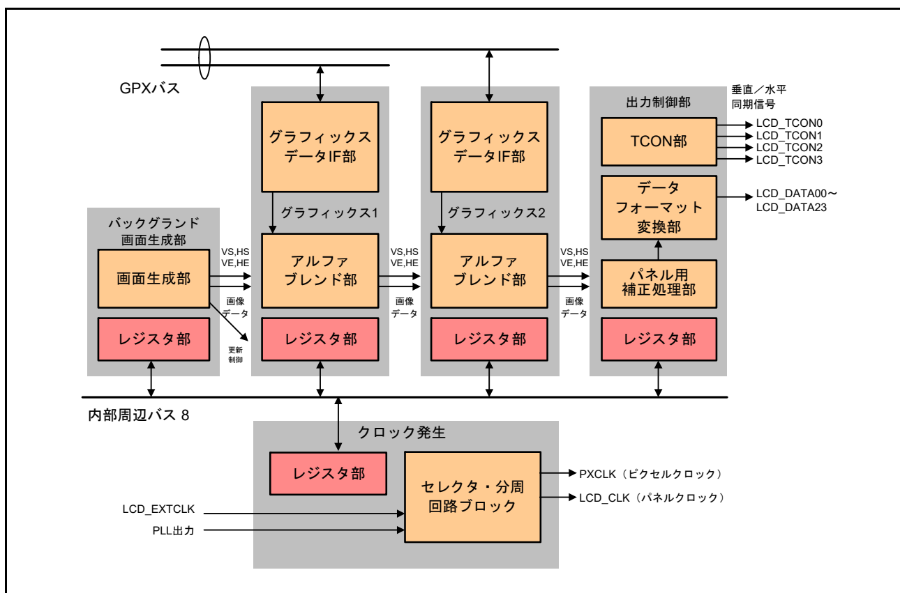
図 58.1 GLCDC のブロック図
