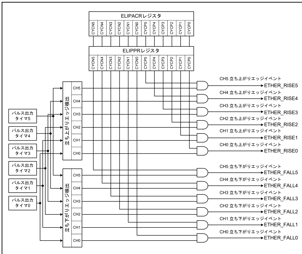
図 30.34 パルス出力タイマと ELC の関係
