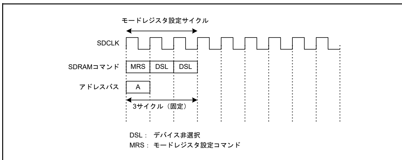
図 15.50 モードレジスタ設定動作タイミング
