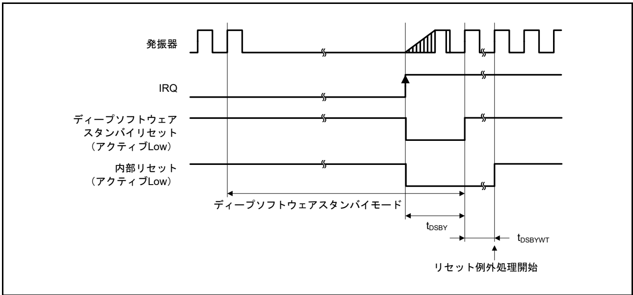
図 60.16 ディープソフトウェアスタンバイモード解除タイミング
