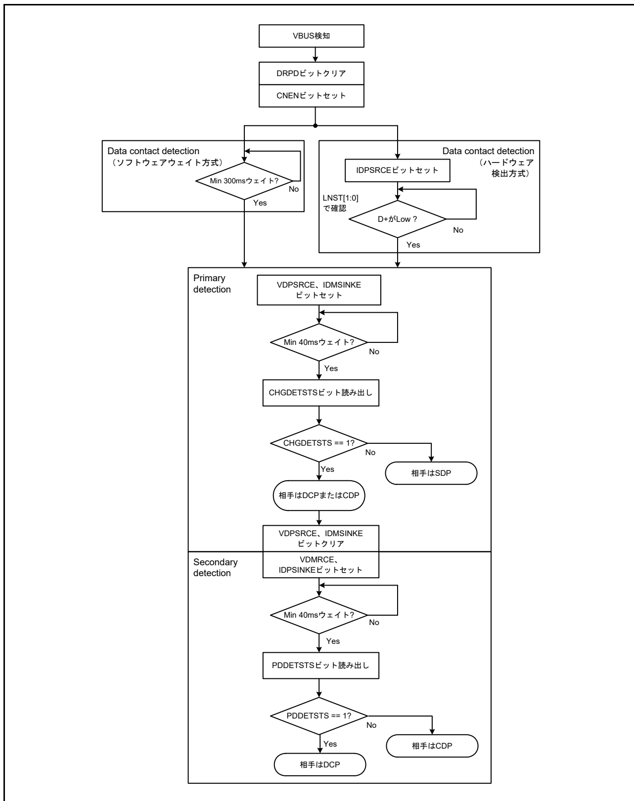
図 33.19 Portable Device としての処理フロー
