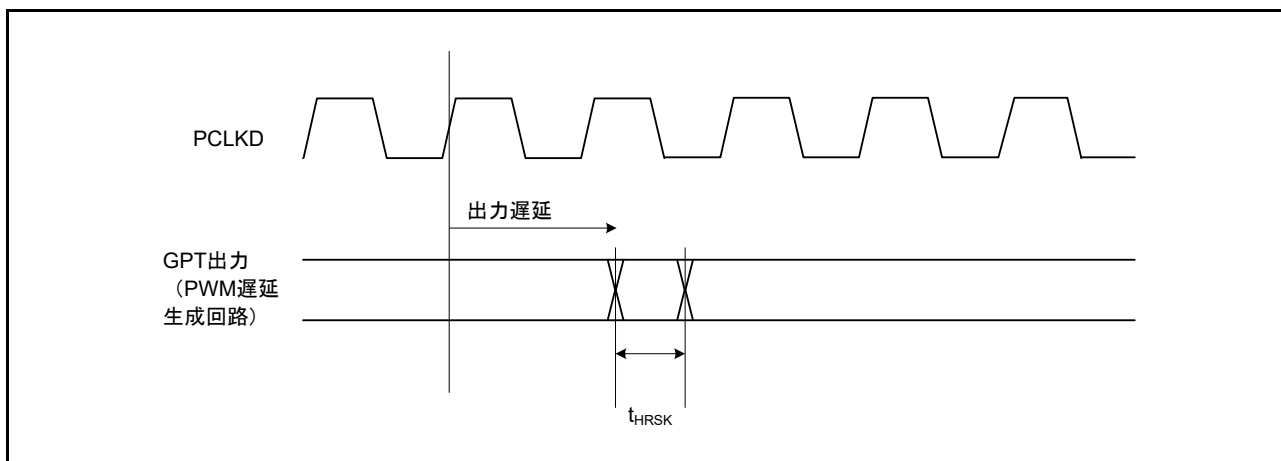
図 60.39 GPT (PWM 遅延生成回路) 出力遅延スキュー
