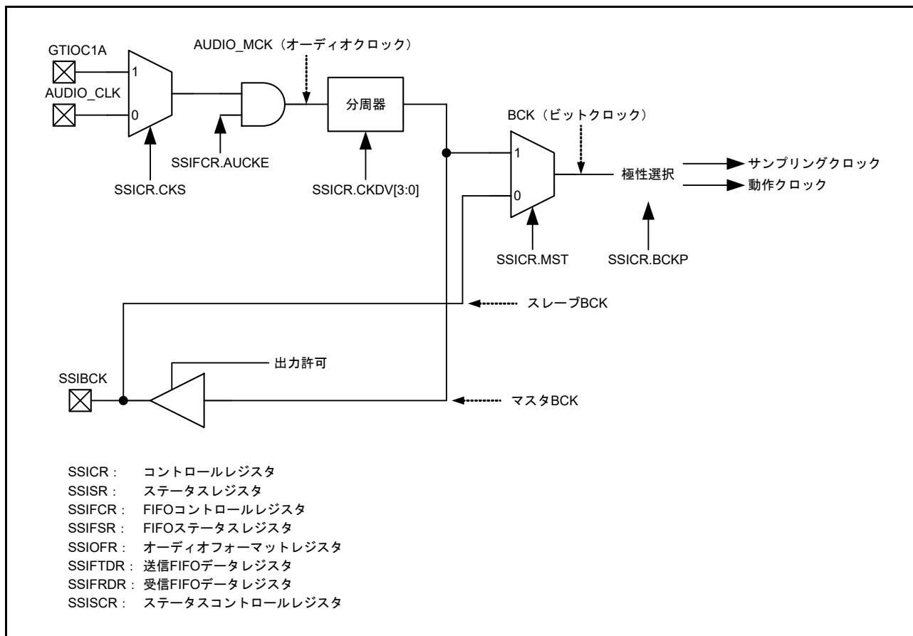
図 41.4 SSIE クロック構成
