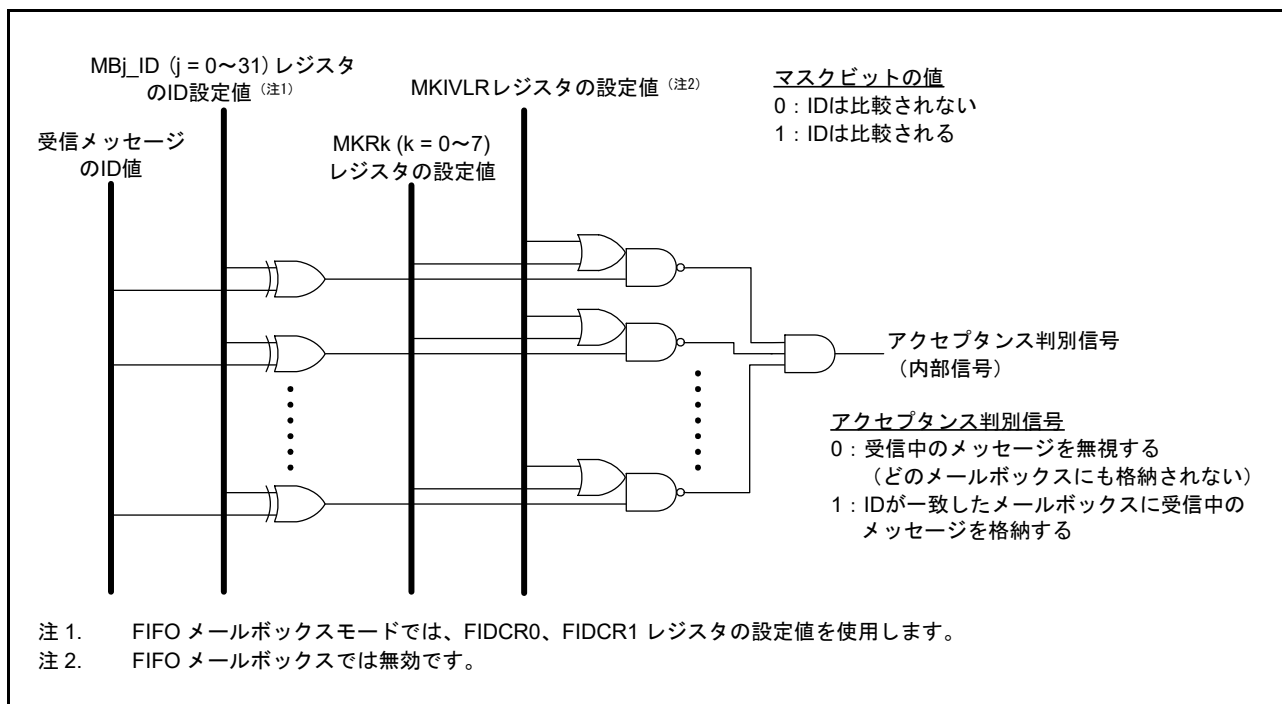
図 37.17 アクセプタンスフィルタ機能
