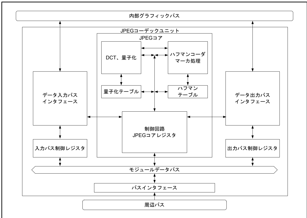
図 57.1 JPEGコーデックのブロック図
