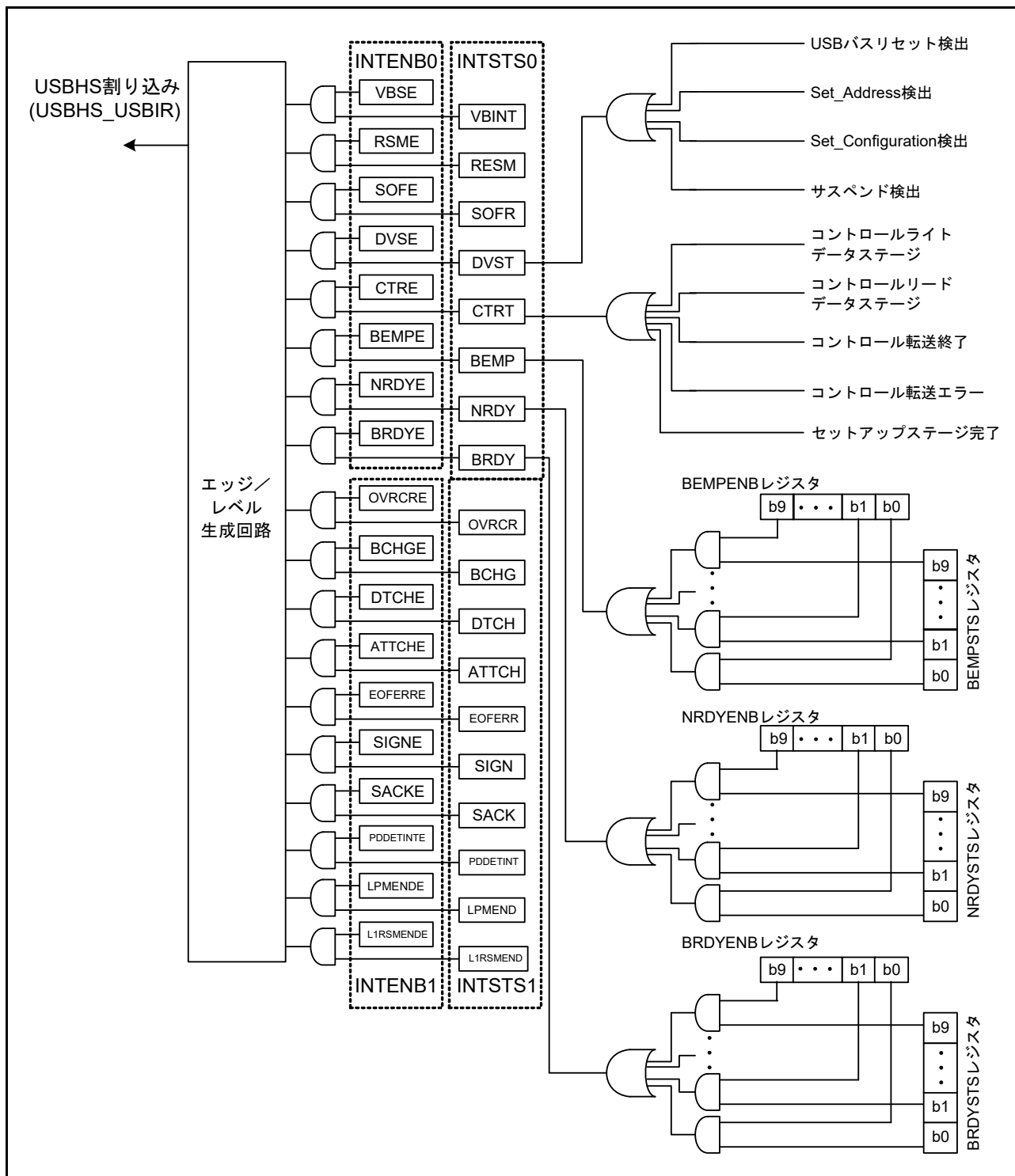
図 33.4 USBHS 割り込み関連回路
