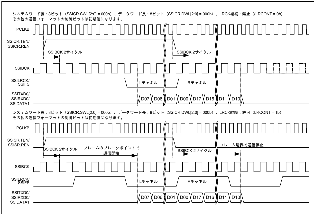
図 41.33 LR クロック/フレーム同期継続の動作例
