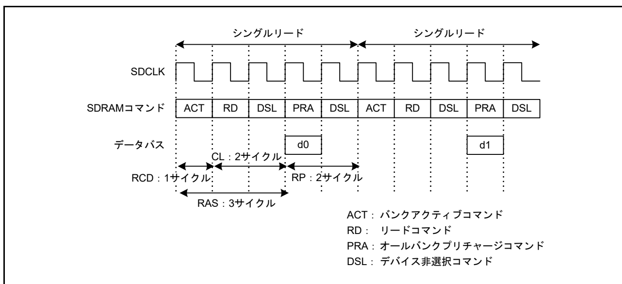
図 15.54 シングルリードタイミング例 (1)
