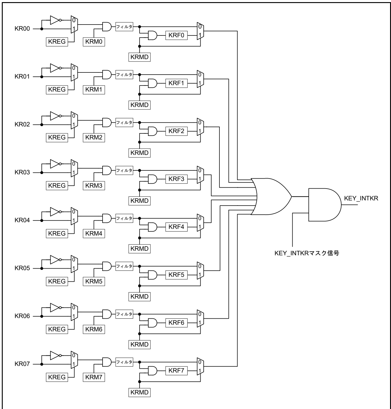
図 21.1 キー割り込みのブロック図
