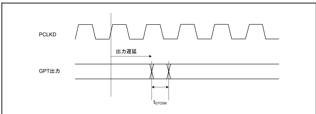
図 60.38 OPS の GPT 出力遅延スキュー
