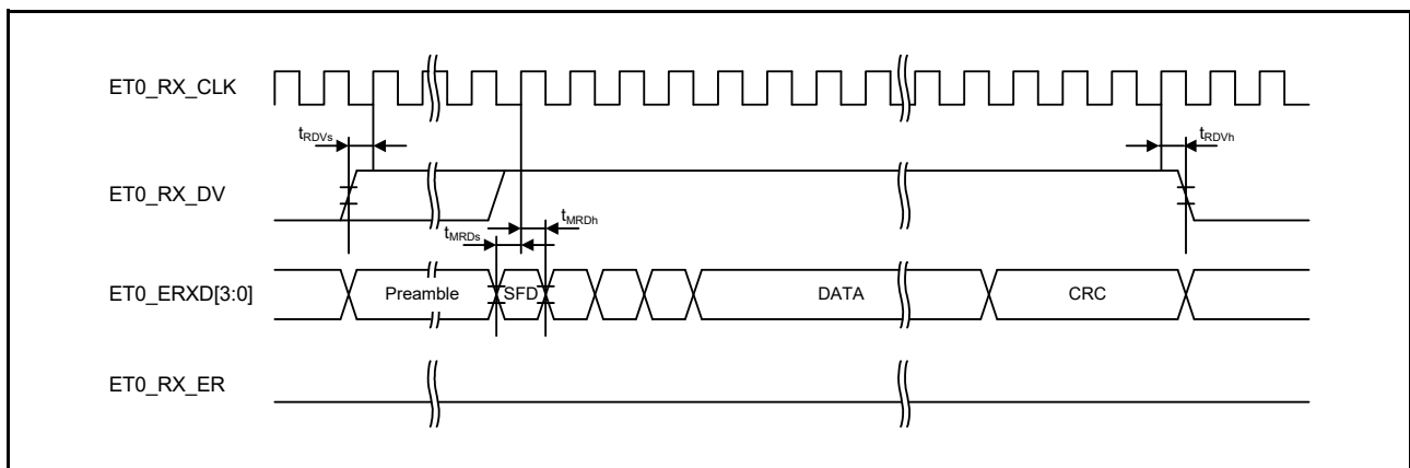
図 60.74 正常動作時の MII 受信タイミング
