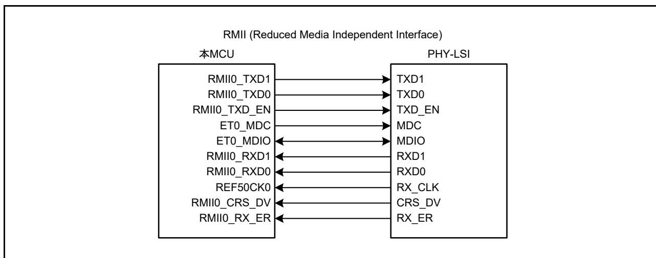
図 29.3 PHY-LSI との接続例 (RMII)
