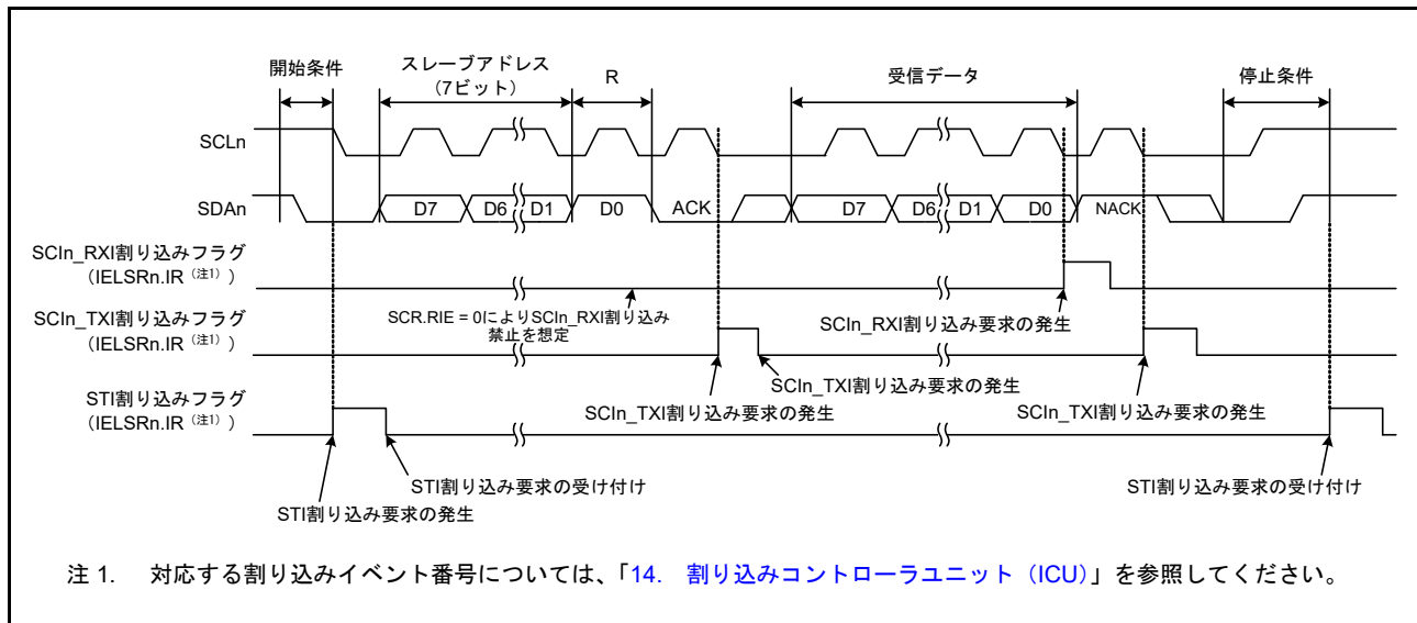
図 34.67 簡易 IIC モードにおけるマスタ受信の動作例 (7 ビットスレーブアドレス、送信割り込み、受信割り込み使用時)
