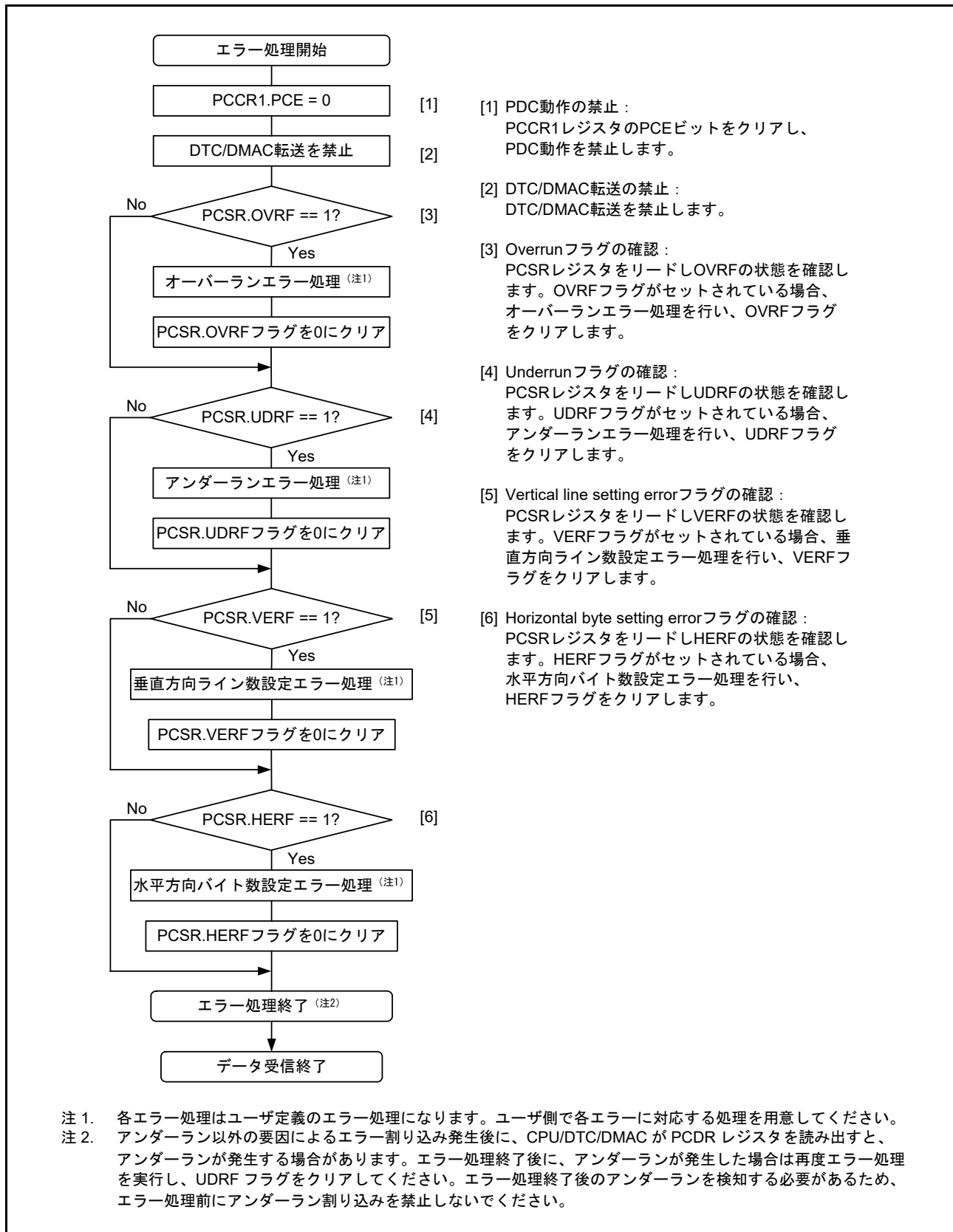
図 44.20 エラー処理フロー例
