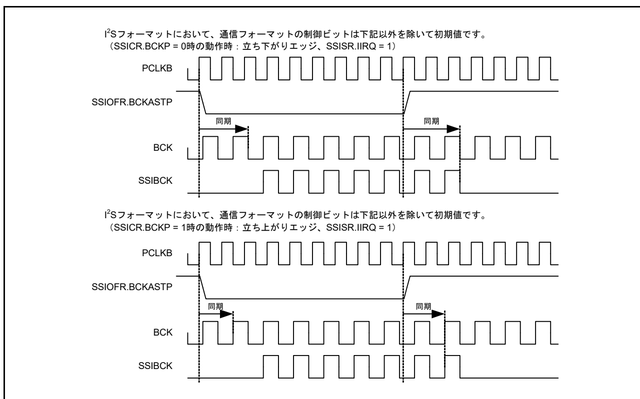
図 41.45 SSIOFR.BCKASTP ビットによる SSIBCK 出力の停止例
