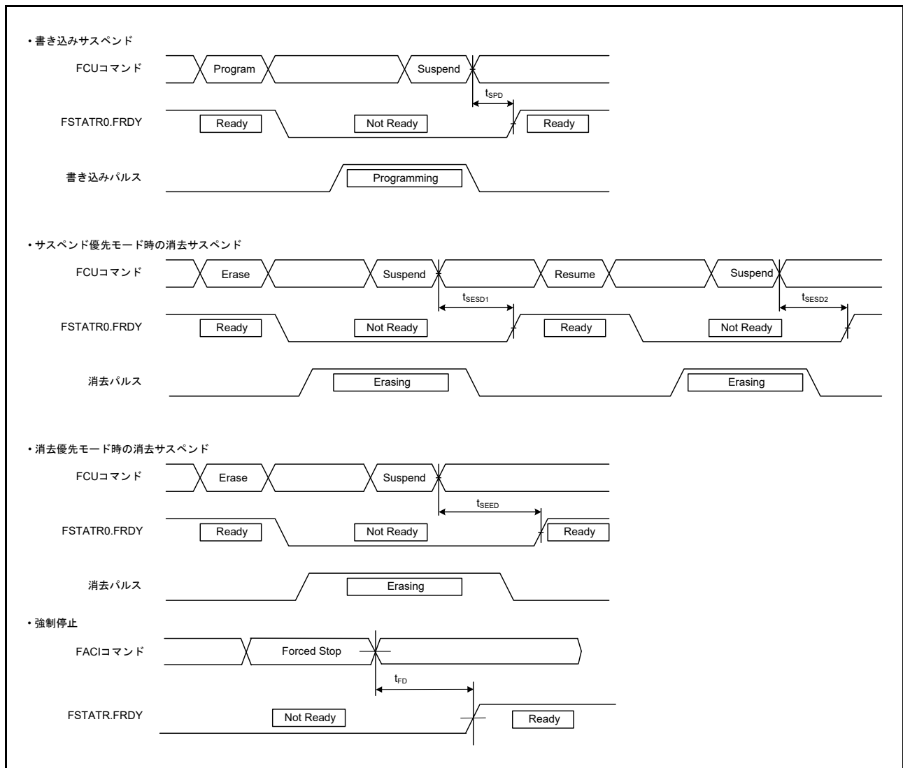
図 60.102 フラッシュメモリのプログラム/イレースのサスペンドタイミングと強制停止タイミング
