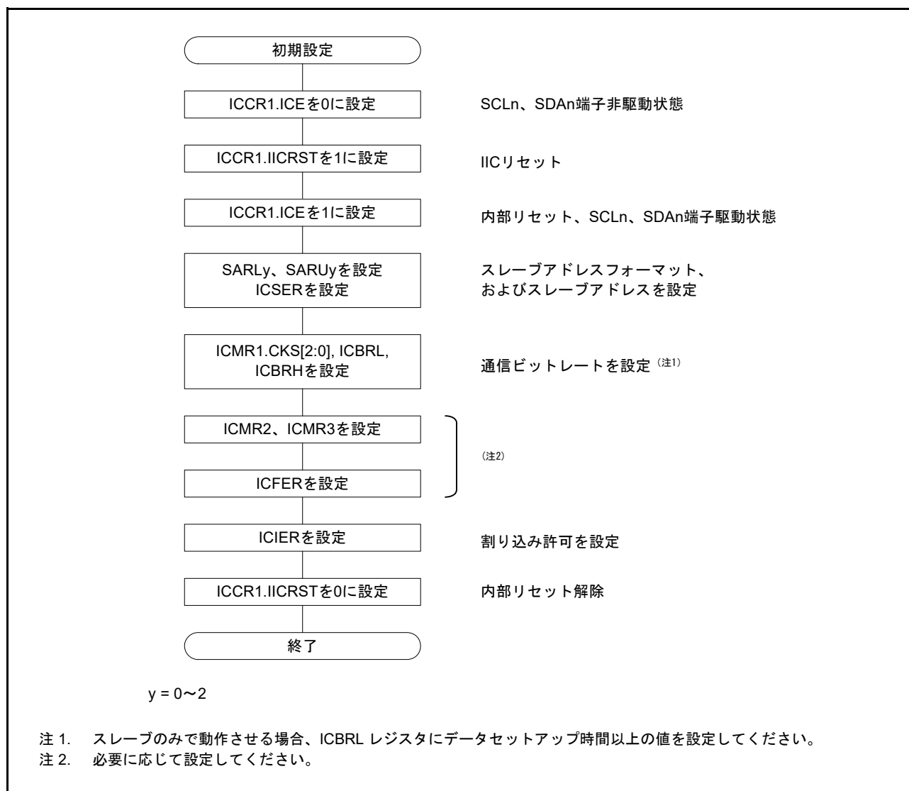
図 36.5 IIC の初期化フローチャート例
