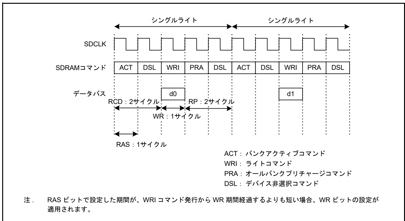
図 15.60 シングルライトタイミング例 (2)
