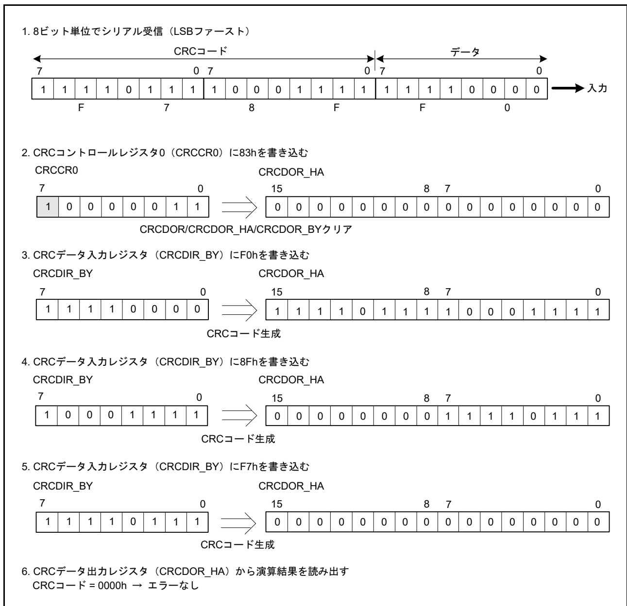
図 40.4 LSB ファーストのデータ受信
