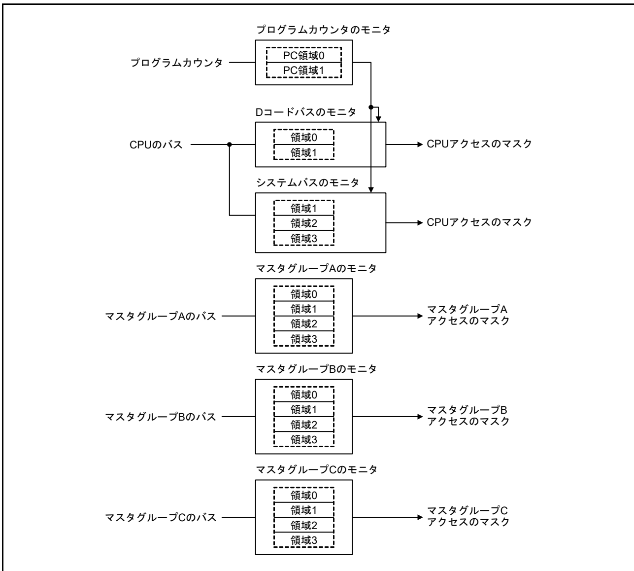
図 16.10 セキュリティ MPU のブロック図
