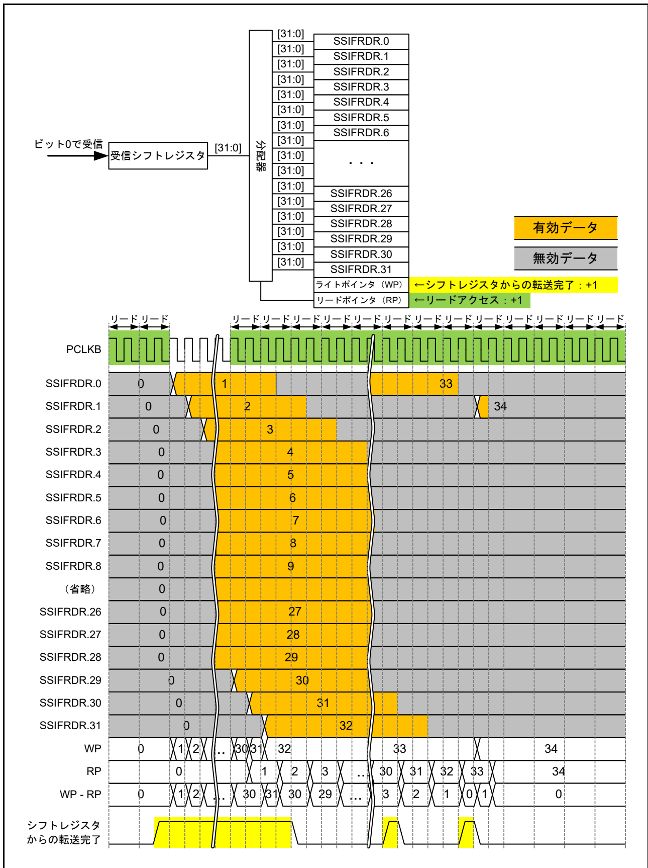
図 41.32 受信 FIFO データレジスタと受信シフトレジスタの構成および FIFO 動作例
