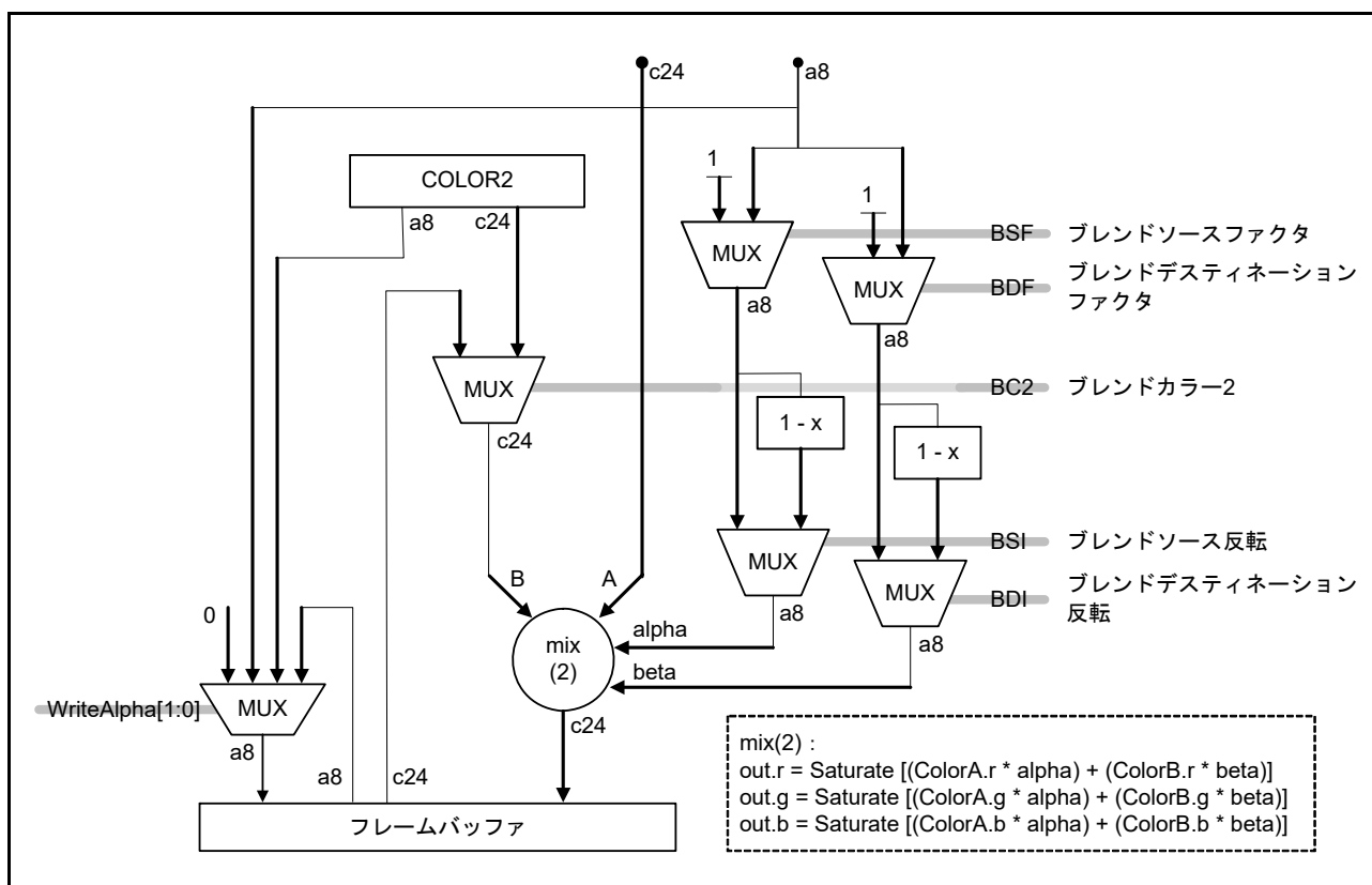
図 56.23 CONTROL2.USEACB = 0 の場合のカラーチャネルブレンドユニット
