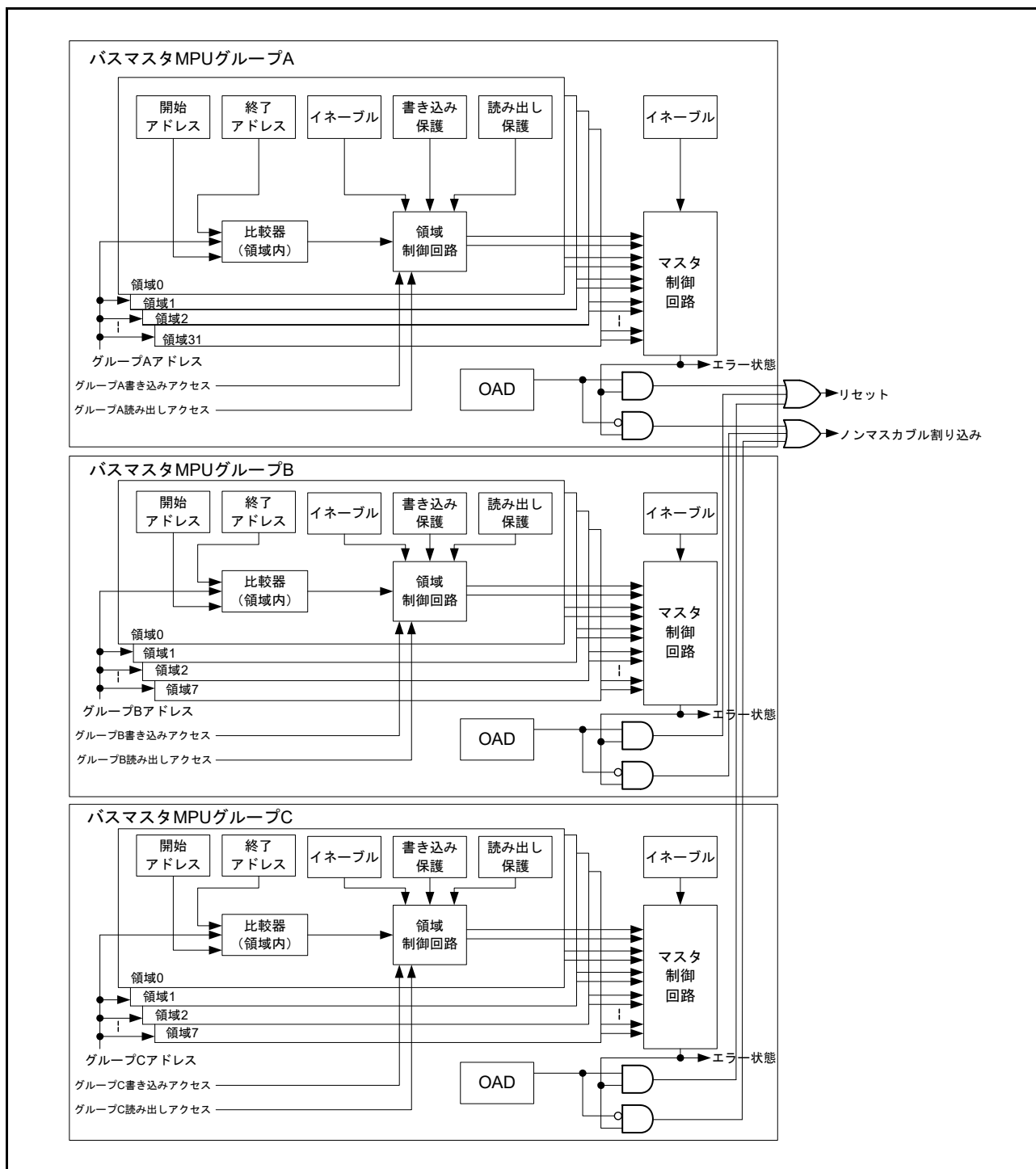
図 16.4 バスマスタ MPU グループ A、B、および C
