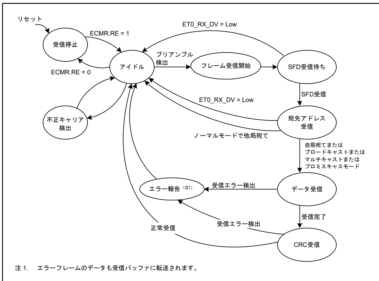
図 29.5 ETHERC 受信部状態遷移図
