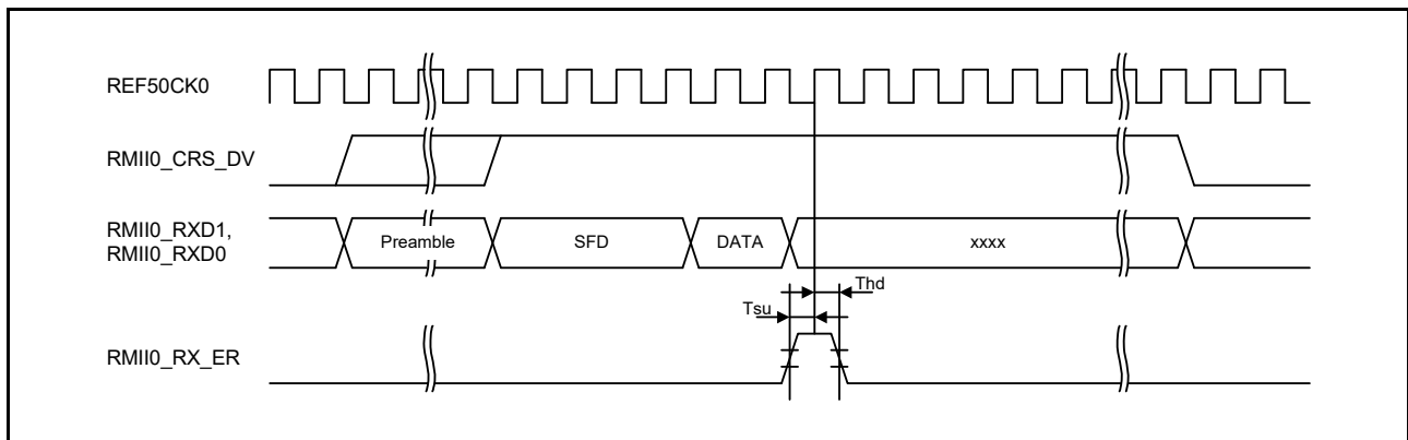
図 60.70 エラー発生時の RMI0 受信タイミング
