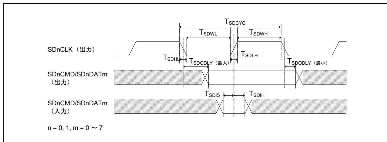
図 60.66 SD/MMC ホストインタフェース信号タイミング
