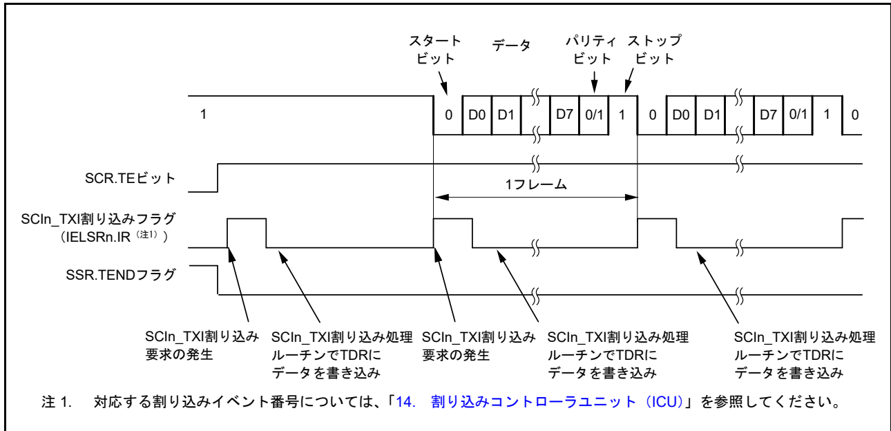
図 34.9 調歩同期式モードにおけるシリアル送信の動作例 (1) (8 ビットデータ/パリティあり/1ストップビット/CTS 機能不使用/送信開始時)
