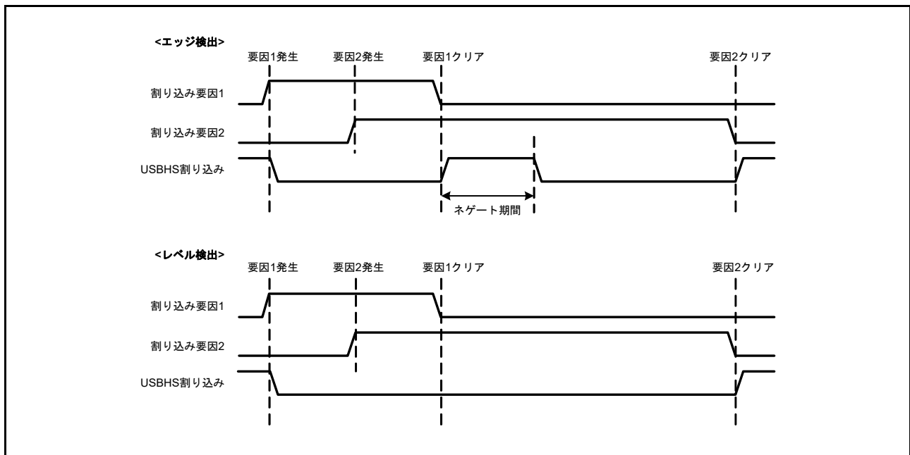
図 33.3 USBHS 割り込み動作
