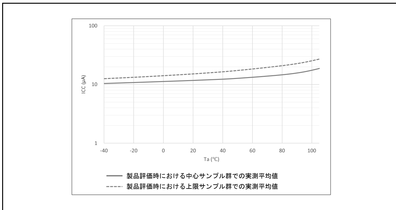
図 60.4 ディープソフトウェアスタンバイモード時に、SRAM または USB レジューム検出部へ電源を供給せず、パワーオンリセット回路の低消費電力機能を無効にする場合の温度依存性（参考データ）
