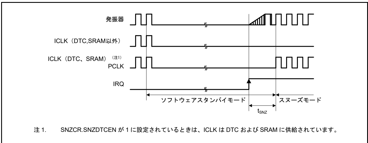
図 60.17 ソフトウェアスタンバイモードからスヌーズモードへのリカバリタイミング
