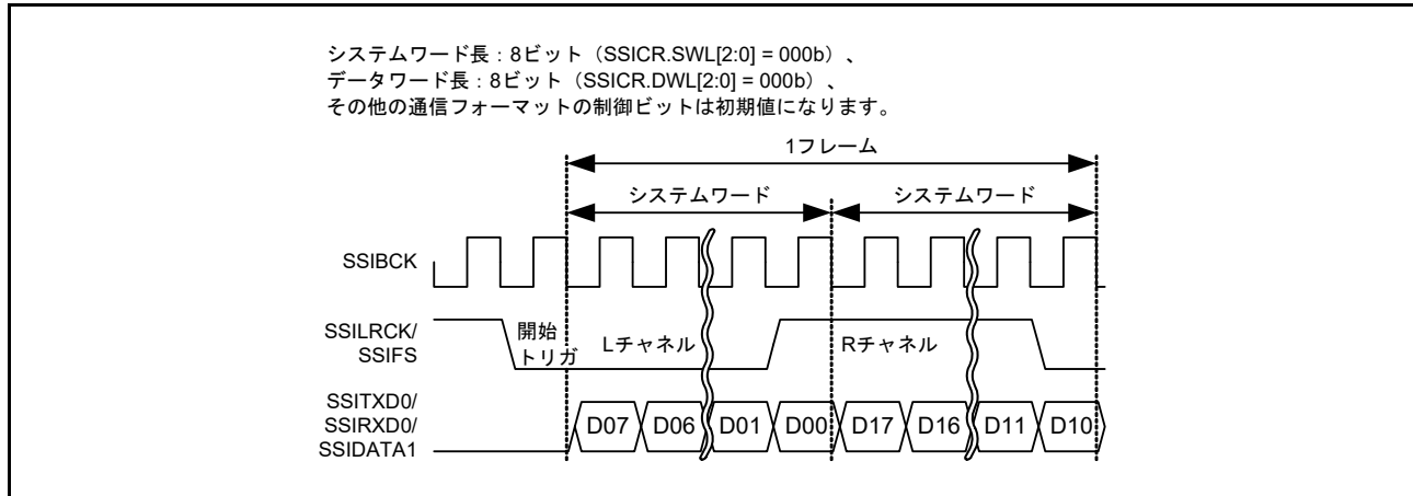
図 41.37 I 2 S フォーマット (パディングなし、システムワード長 = データワード長)
