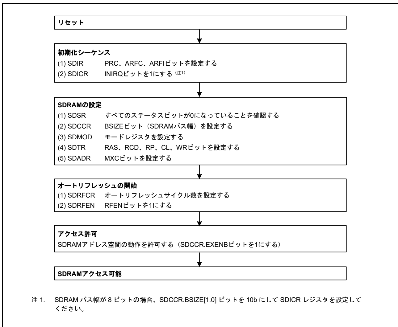
図 15.51 SDRAMC の設定手順
