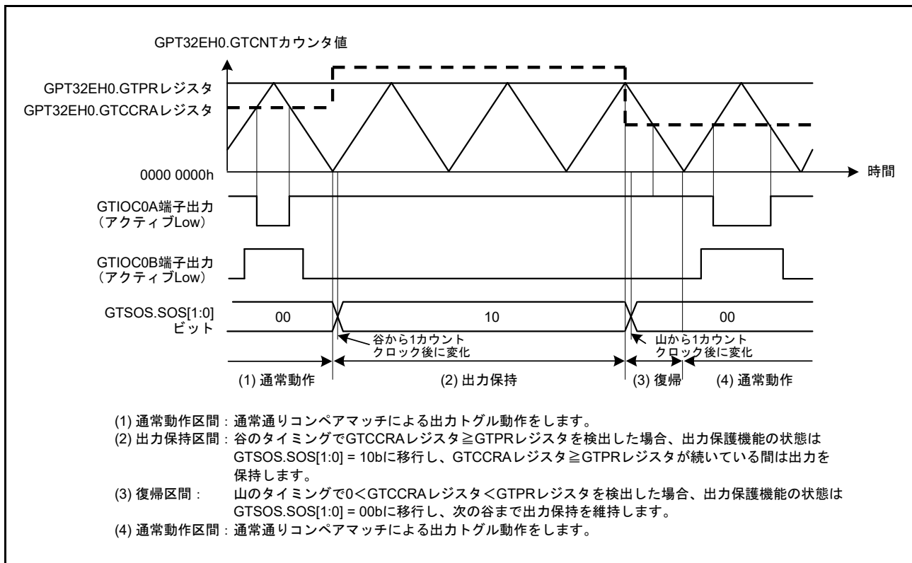
図 23.103 谷でのバッファ転送中に GTCCRA レジスタ \geq GTPR レジスタとなった場合の出力保護機能の動作例 (山でのバッファ転送中に 0 < \text{GTCCRA レジスタ} < \text{GTPR レジスタ} を回復、アクティブ Low の場合)
