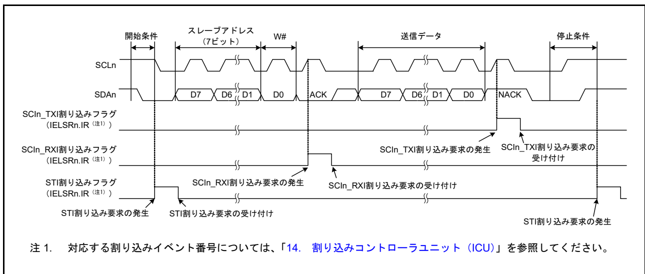
図 34.65 簡易 IIC モードにおけるマスタ送信の動作例 2 (7 ビットスレーブアドレス、ACK 割り込み、NACK 割り込み使用時)
