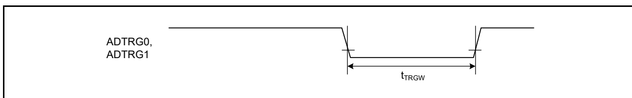
図 60.41 ADC12 トリガ入力タイミング
