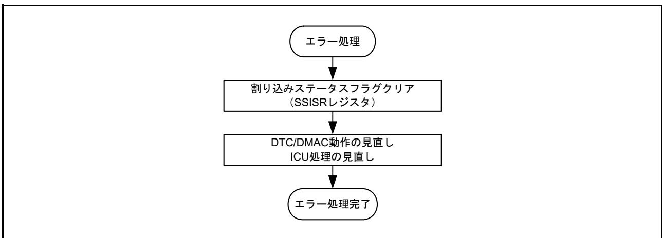
図 41.57 エラー処理手順
