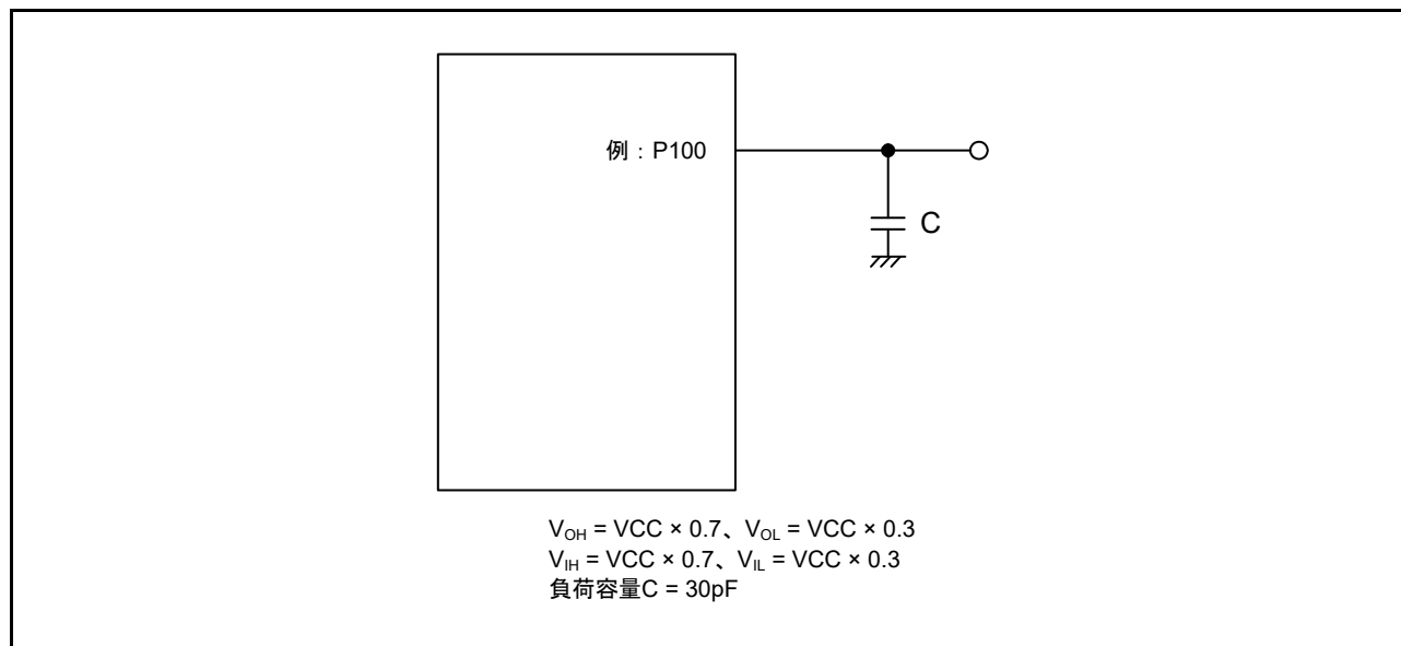
図 60.1 入出力タイミング計測条件
