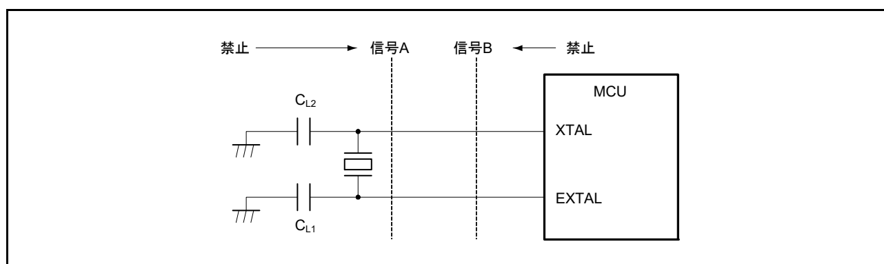
図 9.15 発振回路部のボード設計に関する注意事項 (メインクロック発振器の場合、サブクロック発振器も同様)
