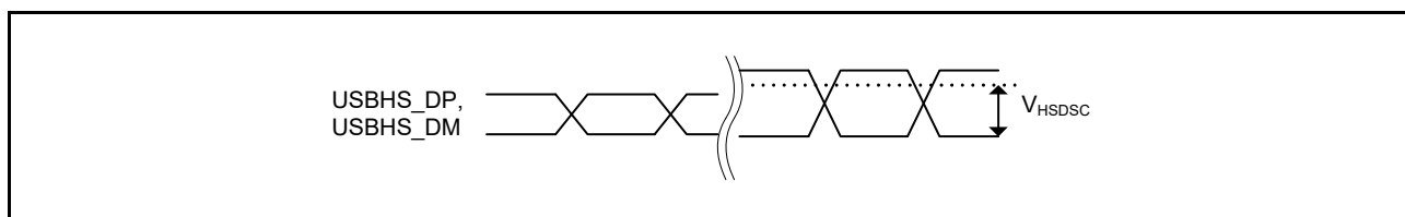
図 60.88 ハイスピードモードにおける USBHS_DP、USBHS_DM の切断検出感度
