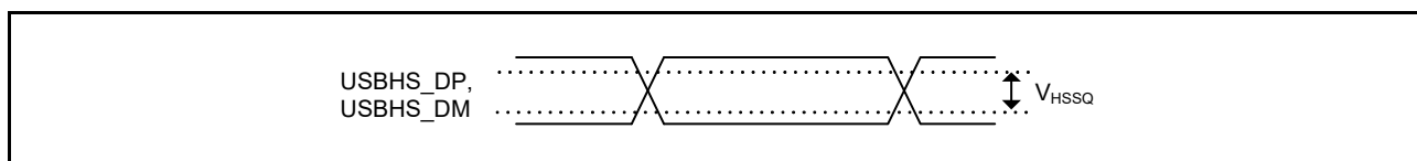
図 60.87 ハイスピードモードにおける USBHS_DP、USBHS_DM の Squelch 検出感度
