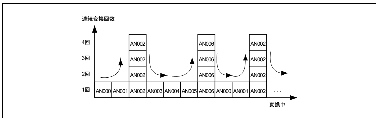
図 47.3 ADADC.ADC[2:0] = 011b、ADADS0.ADS02 = 1、ADS06 = 1 選択時のスキャン変換シーケンス
