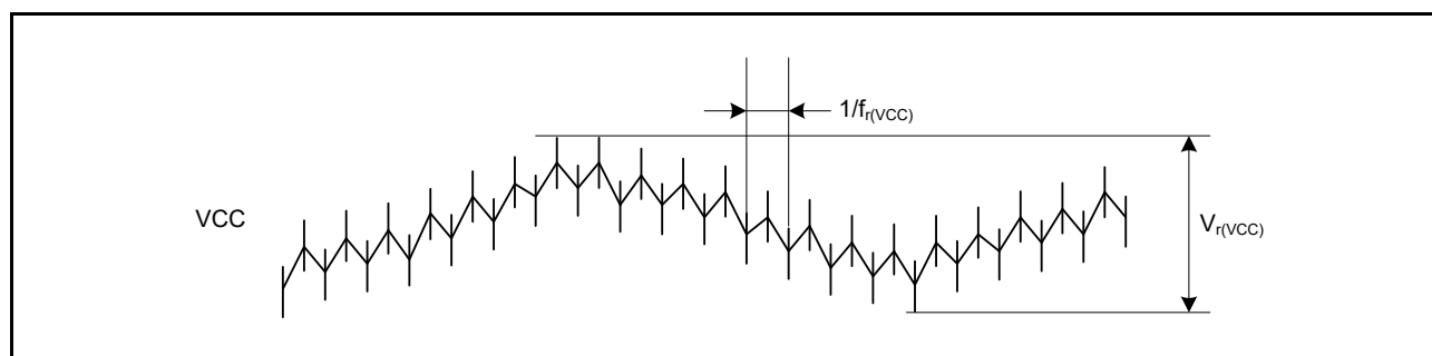
図 60.6 リップル波形
