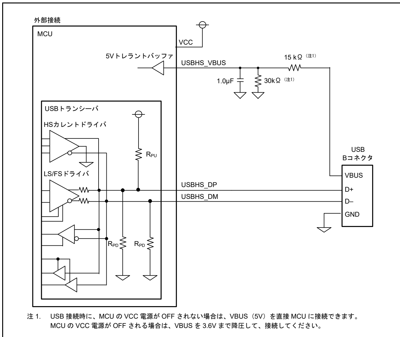
図 33.28 セルフパワーシステムでのデバイス接続例
