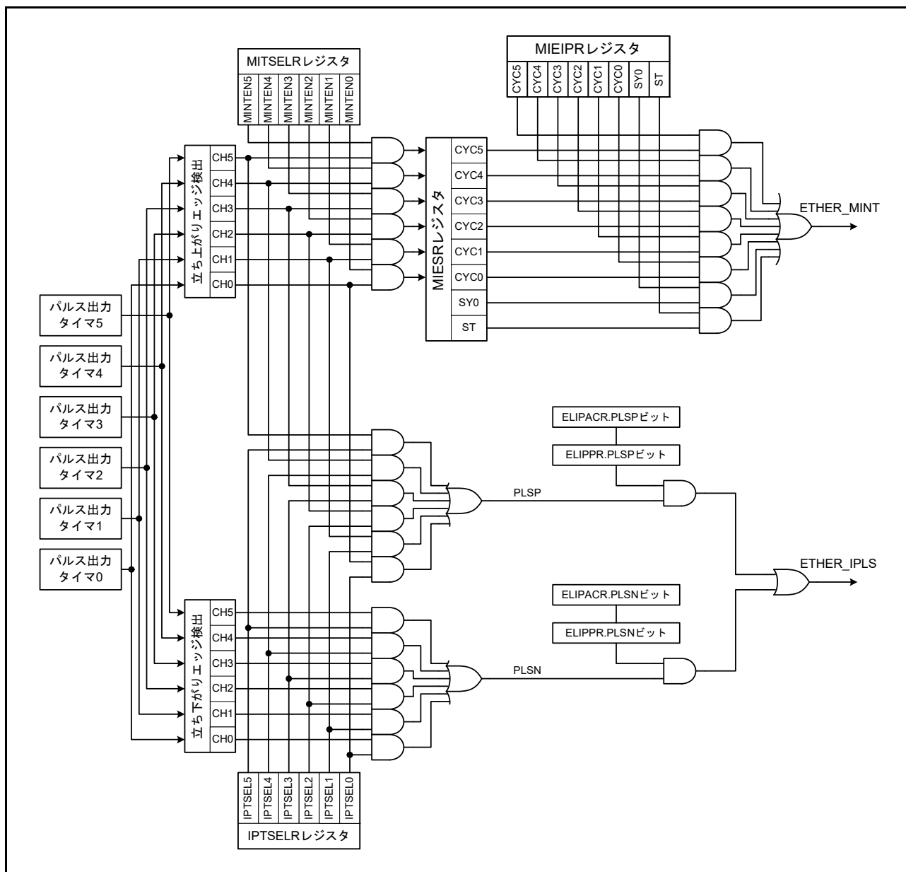
図 30.33 パルス出力タイマの割り込み要求の詳細
