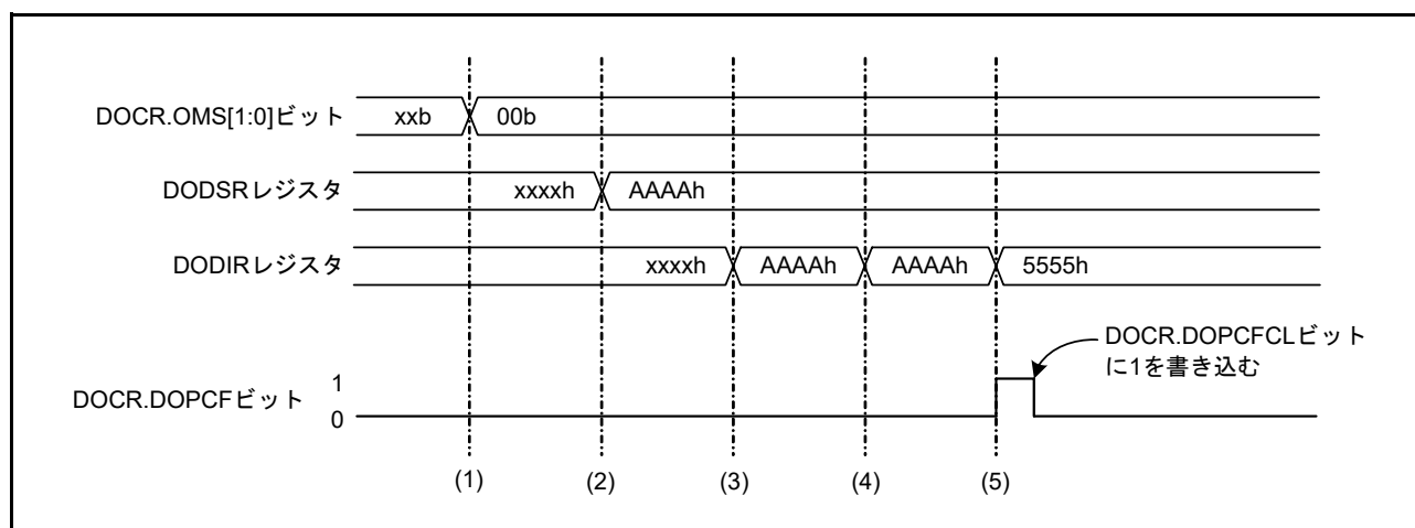
図 52.2 データ比較モードの動作例
