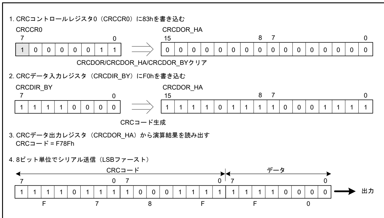
図 40.2 LSB ファーストのデータ送信
