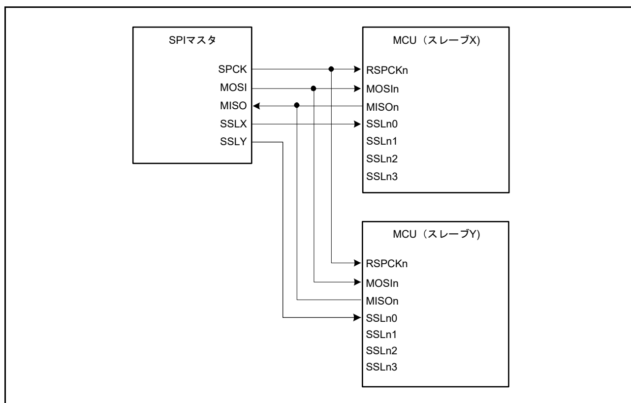
図 38.9 シングルマスタおよびマルチスレーブの構成例 (MCU はスレーブ)
