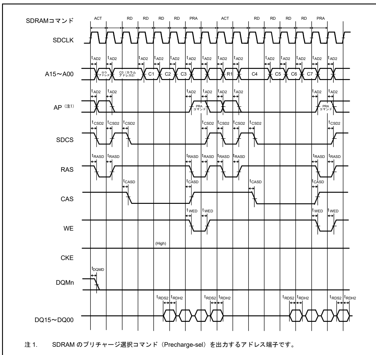
図 60.31 SDRAM 複数リード行またぎタイミング
