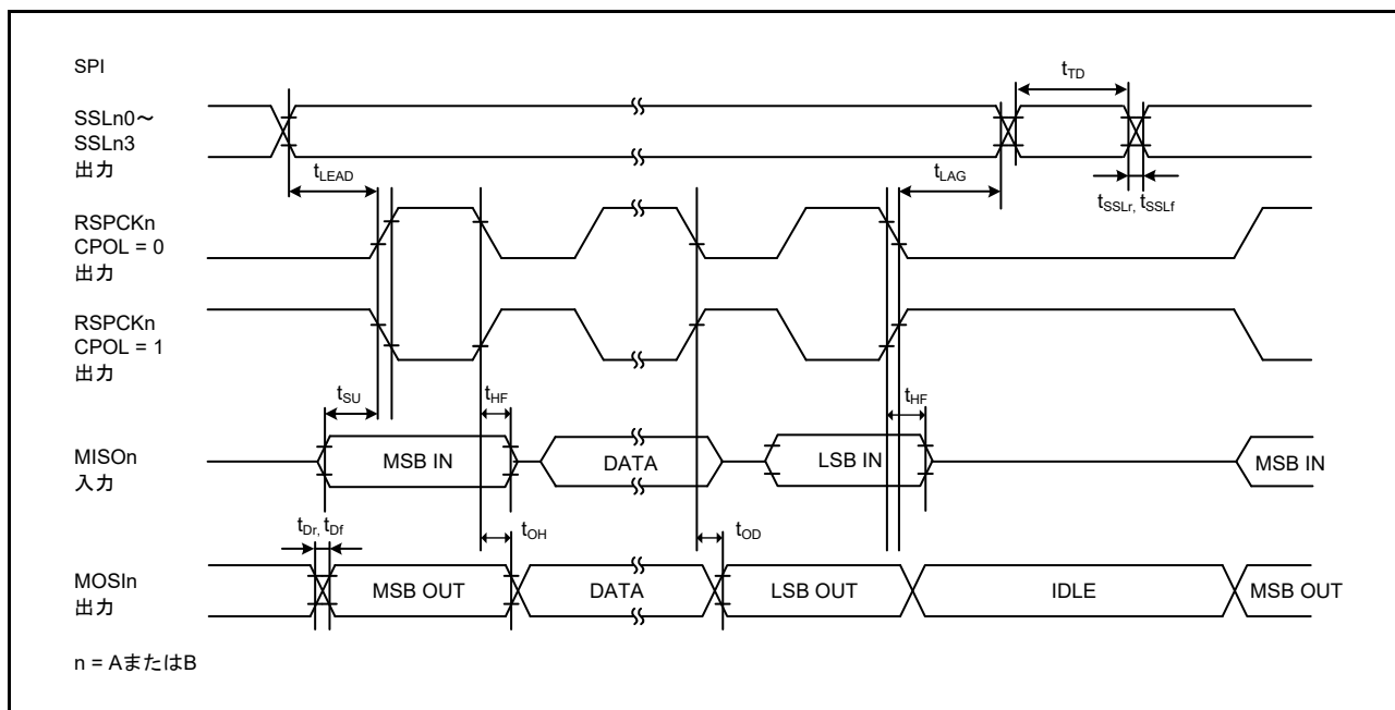
図 60.53 CPHA = 0 で、PCLKA/2 にビットレートが設定されている場合におけるマスタの SPI タイミング
