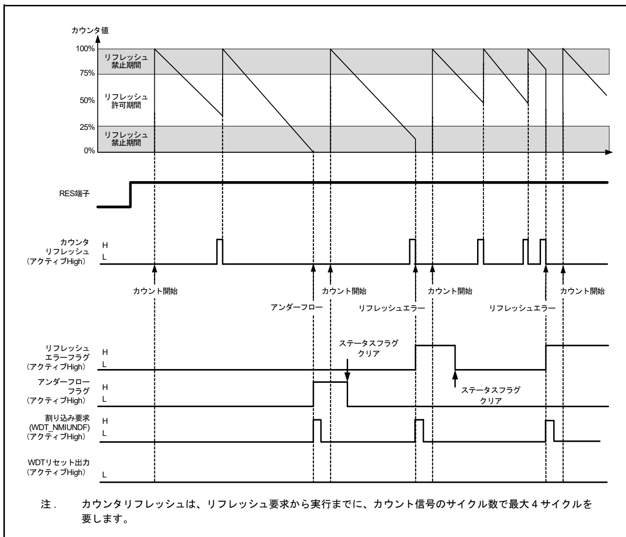
図 27.4 オートスタートモードでの動作例
