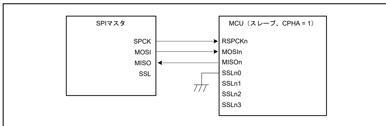
図 38.7 シングルマスタおよびシングルスレーブの構成例 (MCU はスレーブ、CPHA = 1)
