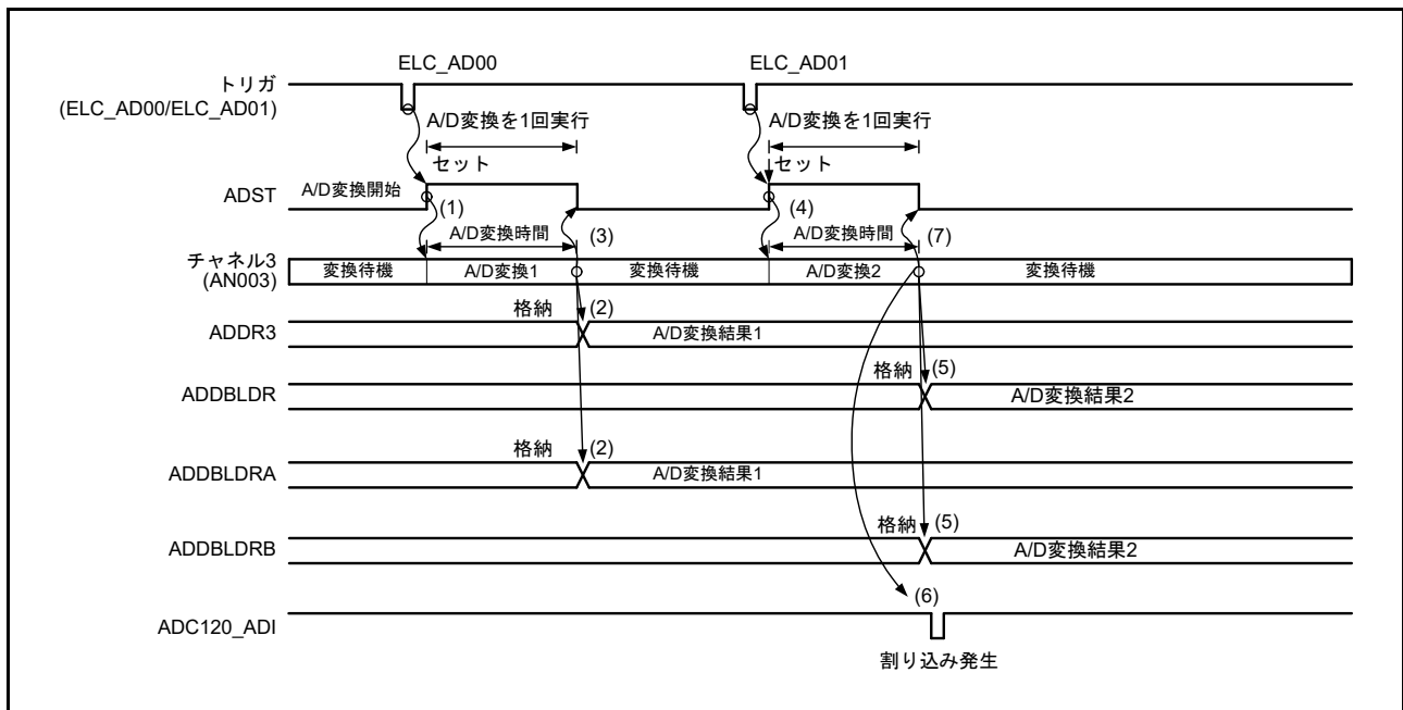
図 47.15 ダブルトリガモードの拡張動作例 (1) (AN003 の 2 重化を選択、ELC_AD00/ELC_AD01 選択)
