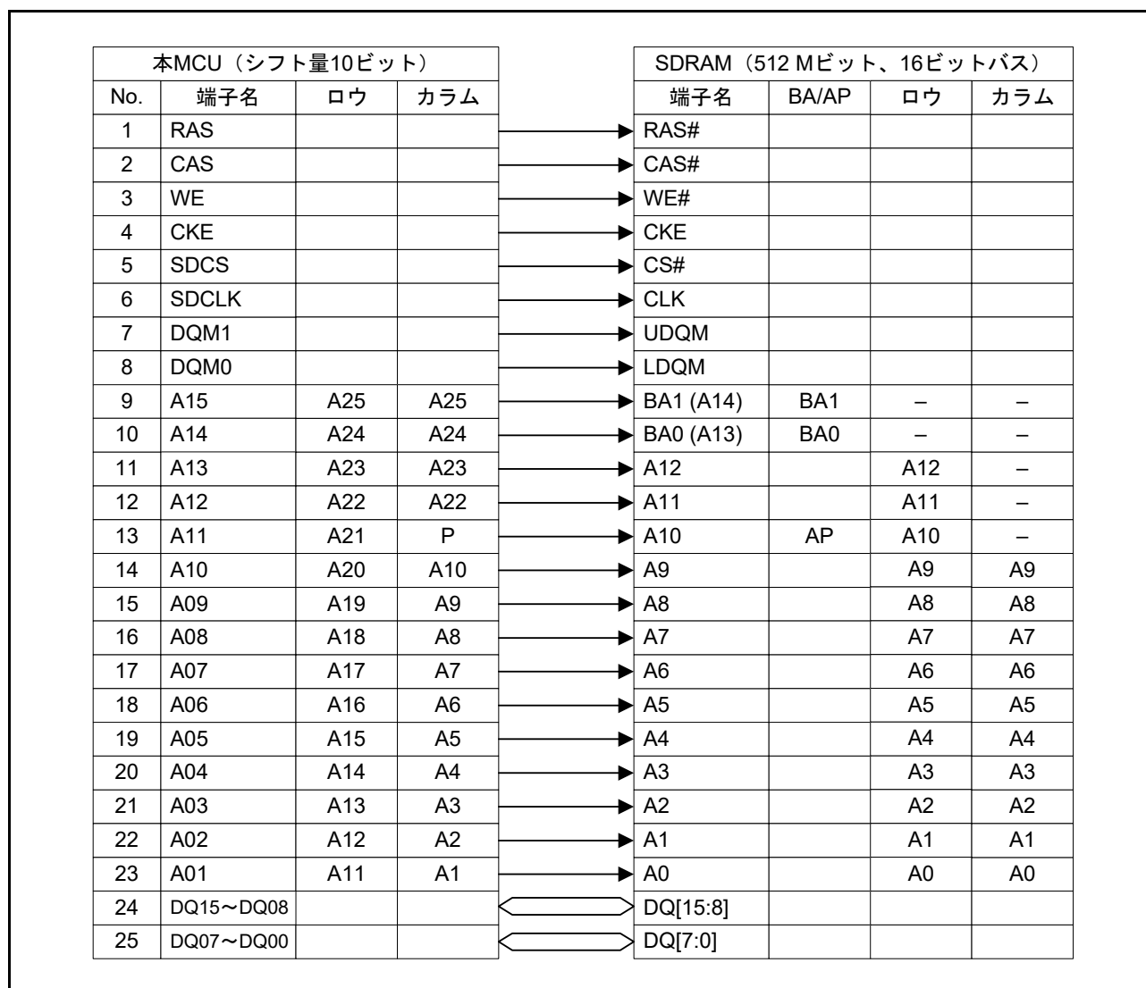
図 15.71 SDRAM 接続例 (512M ビット品 × 1 個、16 ビットバス)
