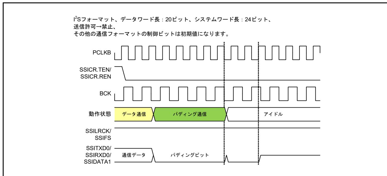
図 41.51 パディング通信からの停止
