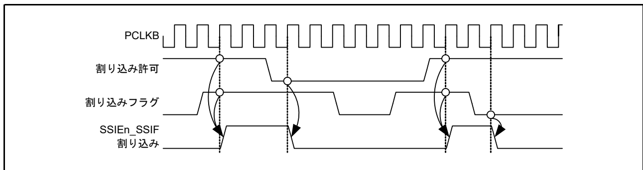
図 41.59 割り込み要因共通のタイミング図 (SSIE n _SSIF)
