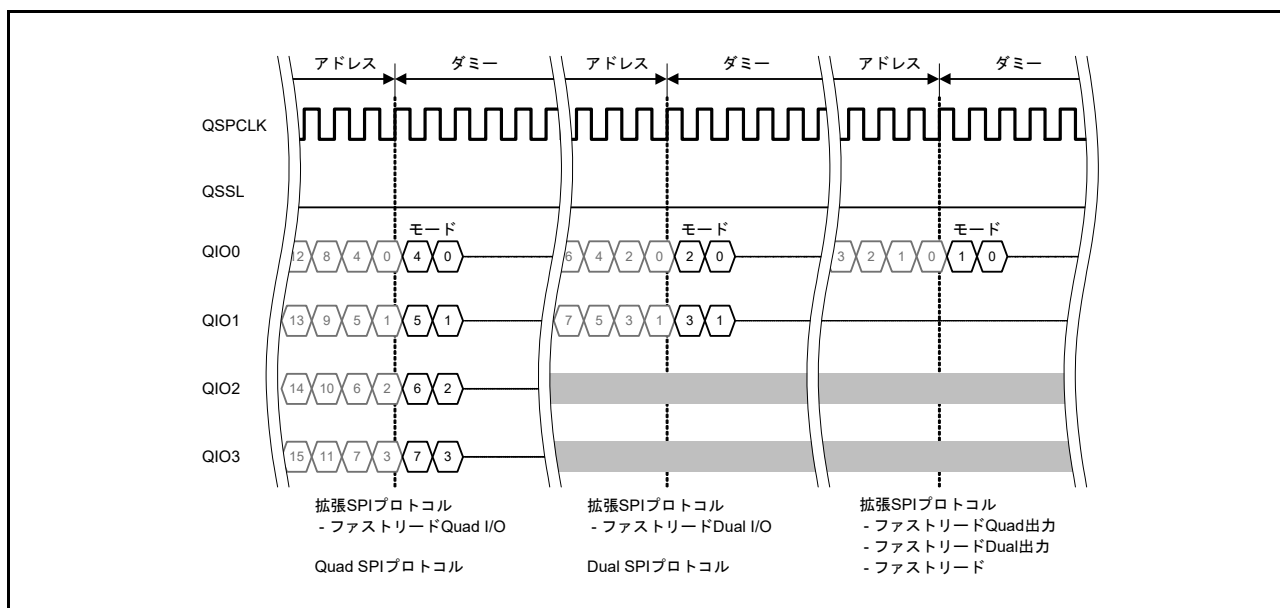
図 39.32 XIP モード制御データ
