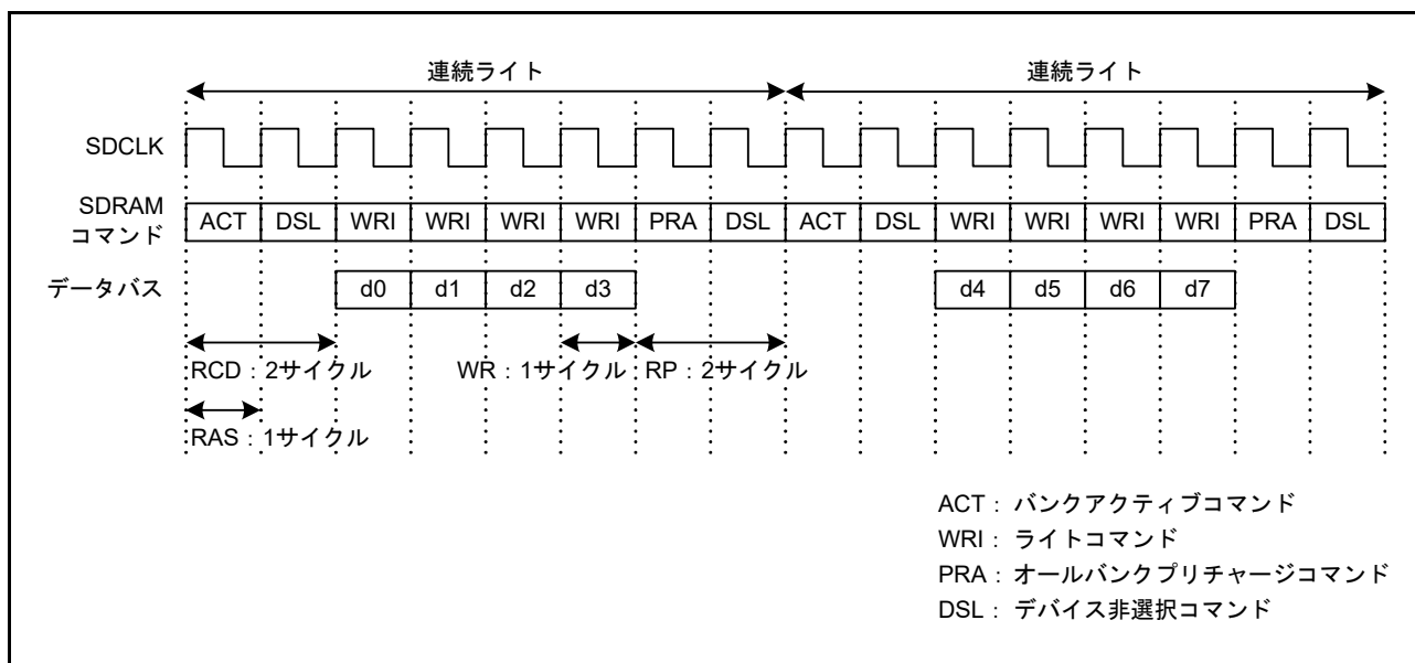
図 15.68 連続ライトタイミング例 (2)
