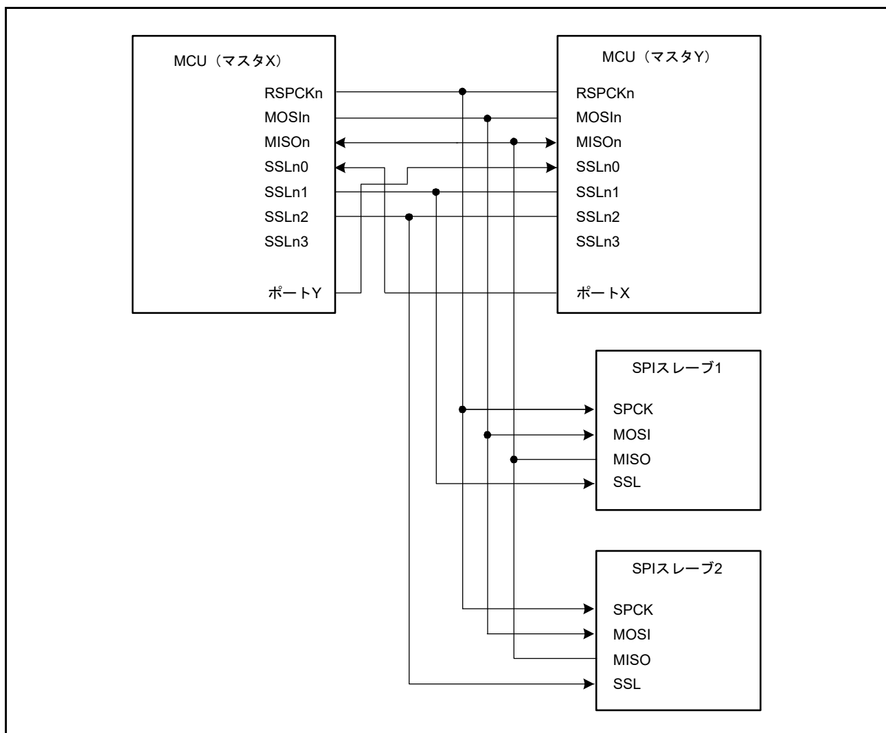
図 38.10 マルチマスタおよびマルチスレーブの構成例 (MCU はマスタ)
