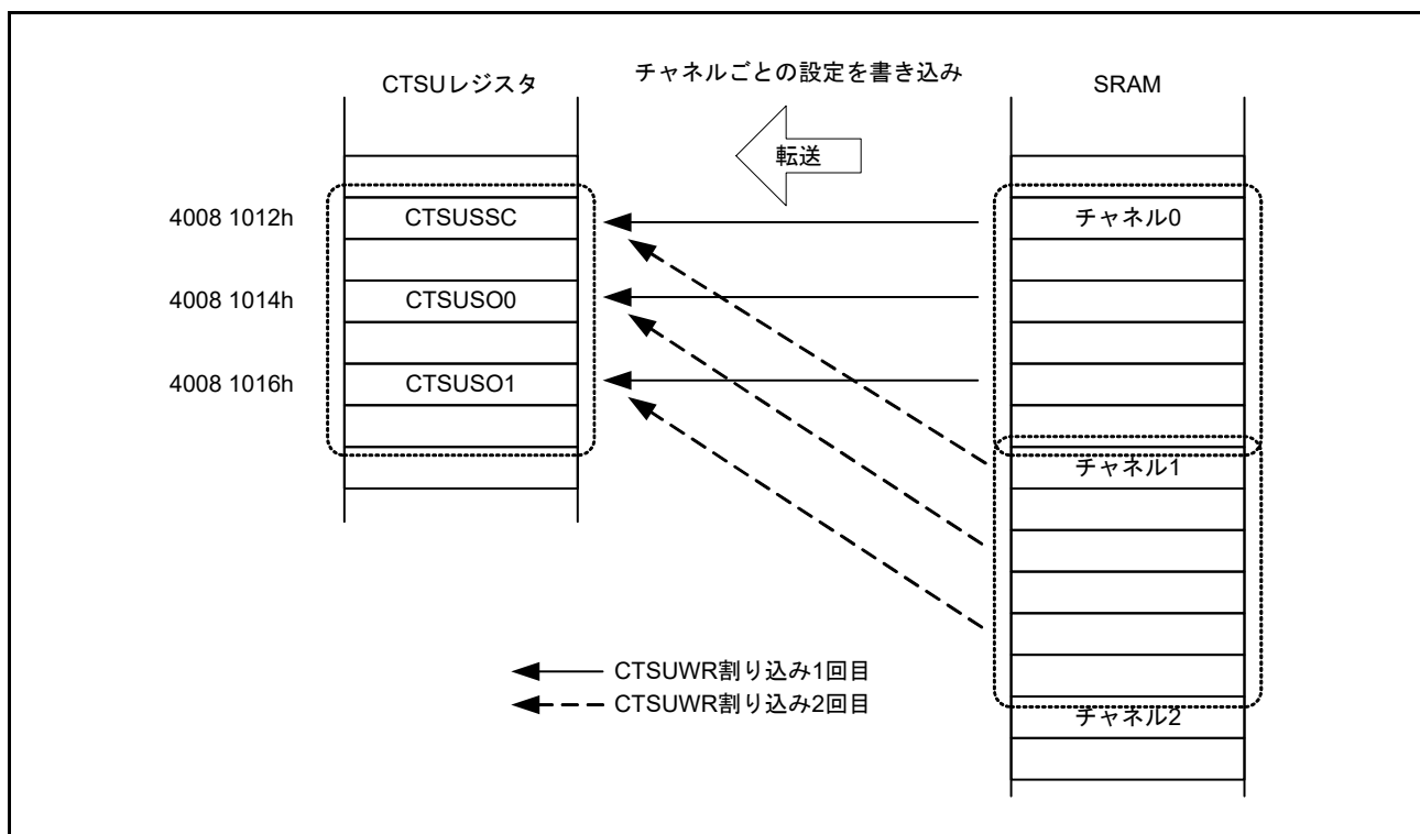
図 51.19 CTSU_CTSUWR 割り込みを用いた DTC 転送動作例
