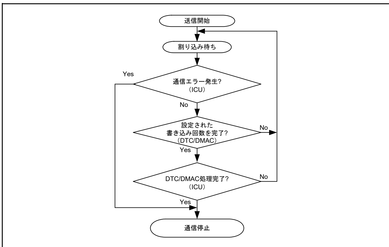
図 41.54 送信手順
