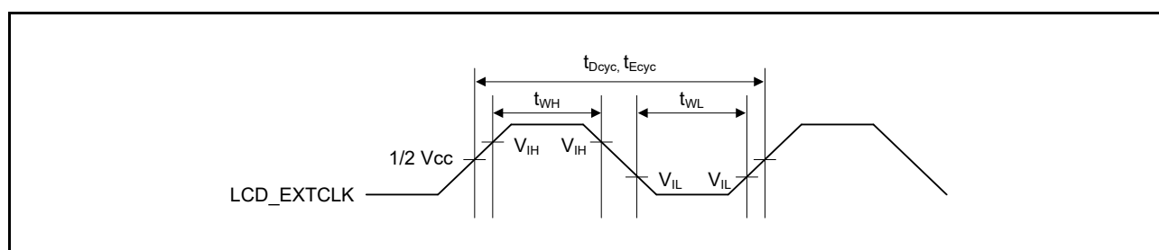
図 60.80 LCD_EXTCLK クロック入カタイミング
