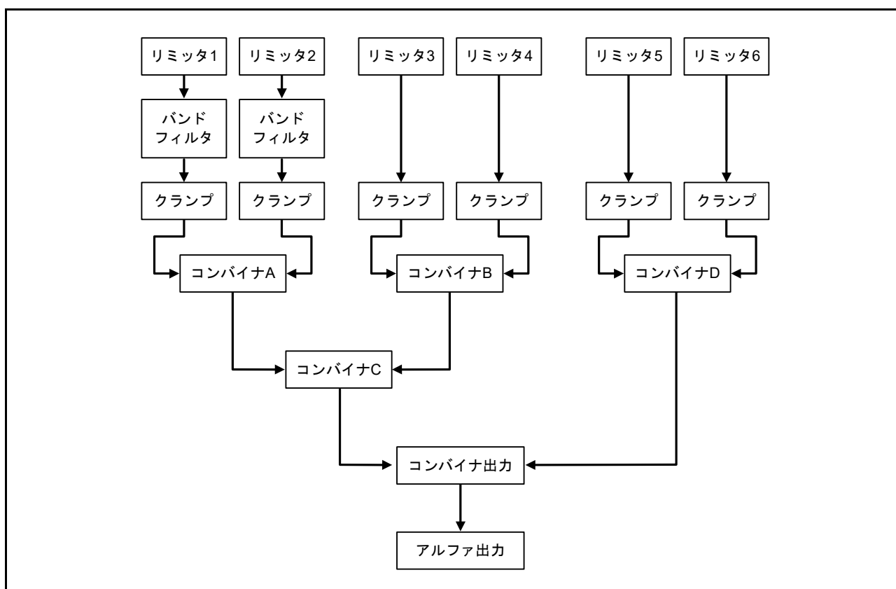
図 56.6 ラスタライゼーションユニットのブロック図
