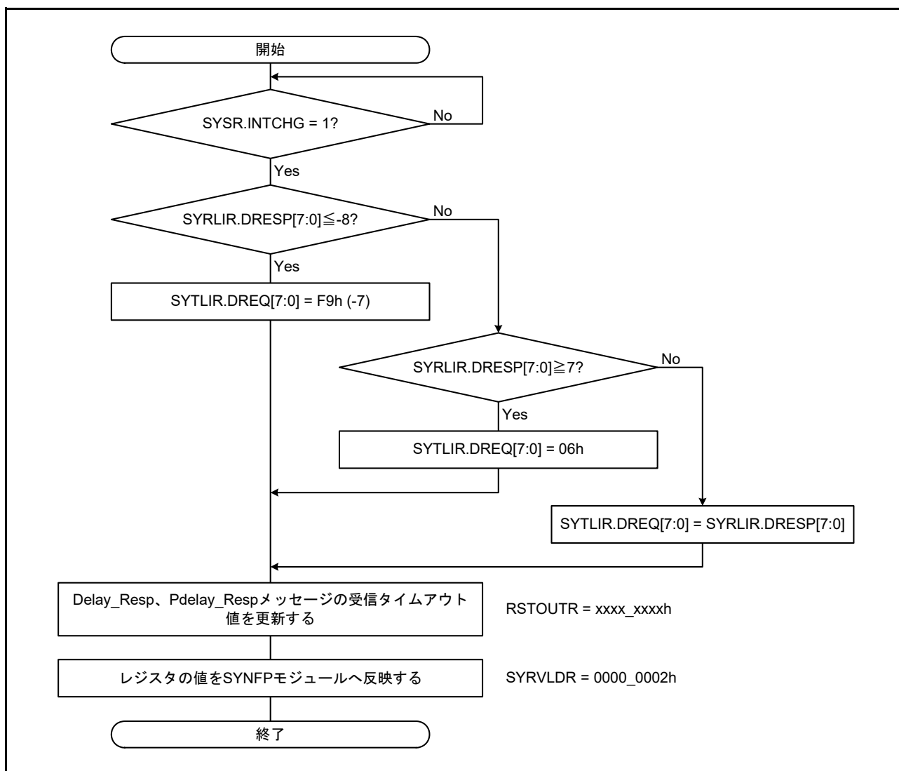
図 30.12 Delay_Req メッセージの送信間隔の変更手順
