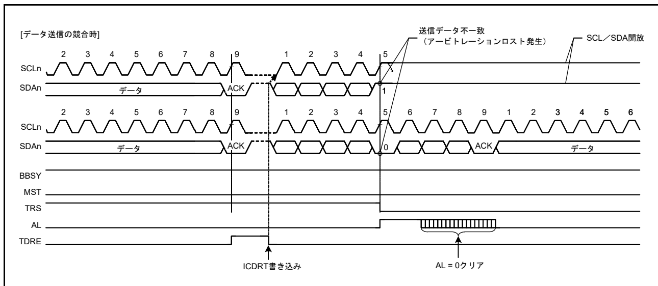
図 36.44 スレーブアービトレーションロスト検出の動作例 (SALE = 1 の場合)
