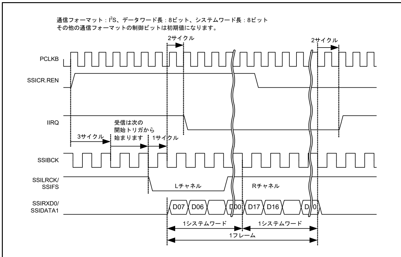
図 41.15 IIRQ 設定タイミング (受信)
