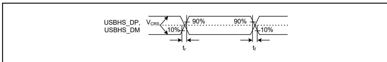
図 60.83 ロースピードモードにおけるUSBHS_DP、USBHS_DMの出力タイミング
