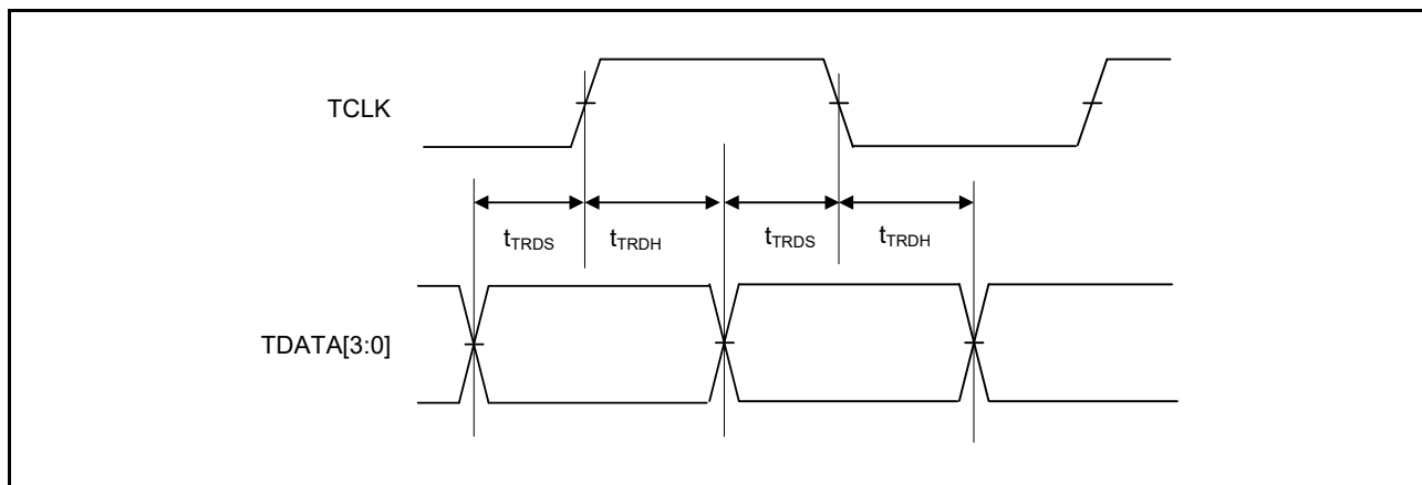
図 60.111 ETM 出力タイミング
