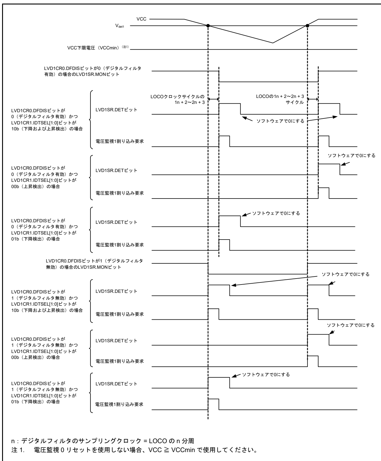
図 8.5 電圧監視 1 割り込みの動作例
