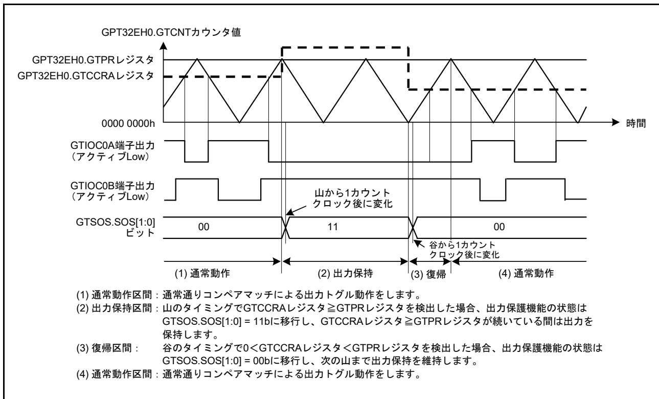
図 23.105 山でのバッファ転送中に GTCCRA レジスタ \geq GTPR レジスタとなった場合の出力保護機能の動作例 (谷でのバッファ転送中に 0 < \text{GTCCRA レジスタ} < \text{GTPR レジスタ} を回復、アクティブ Low の場合)
