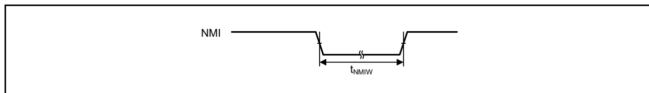
図 60.18 NMI 割り込み入カタイミング
