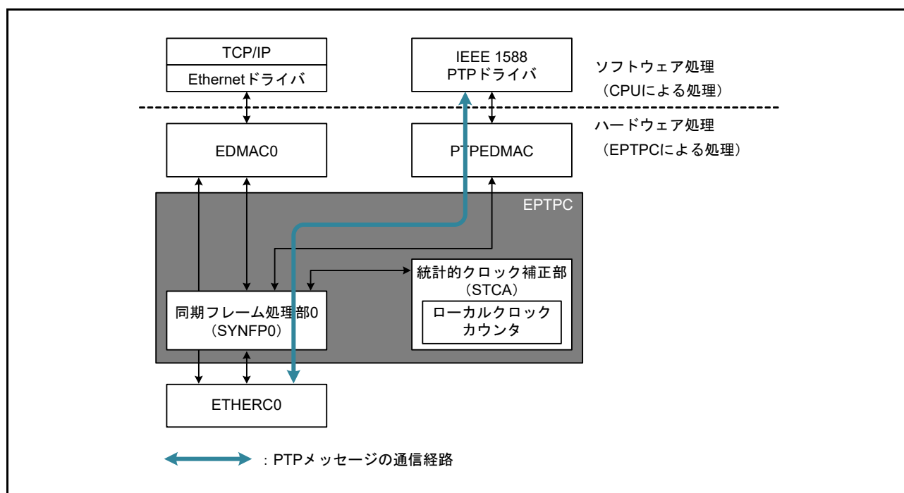
図 30.5 ソフトウェア処理が必要な PTP メッセージの通信経路
