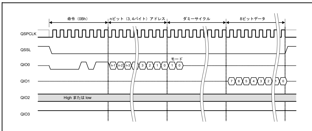
図 39.16 ファストリードバスサイクル
