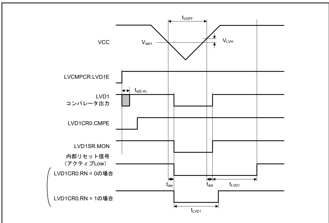
図 60.99 電圧検出回路タイミング ( V_{det1} )
