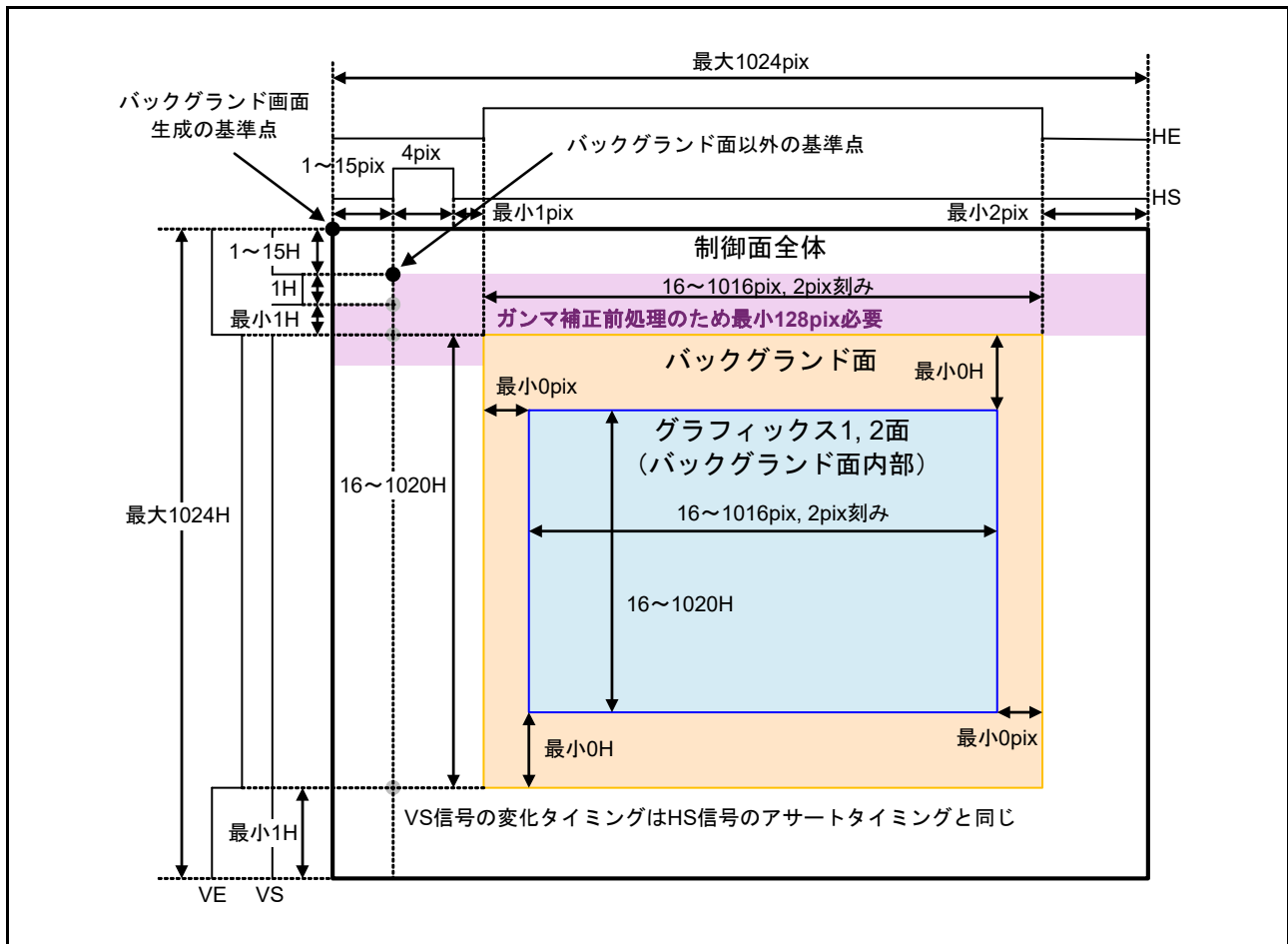
図 58.3 内部画面フォーマット
