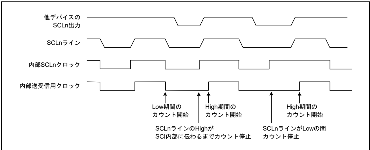
図 34.61 クロック同期化の動作例
