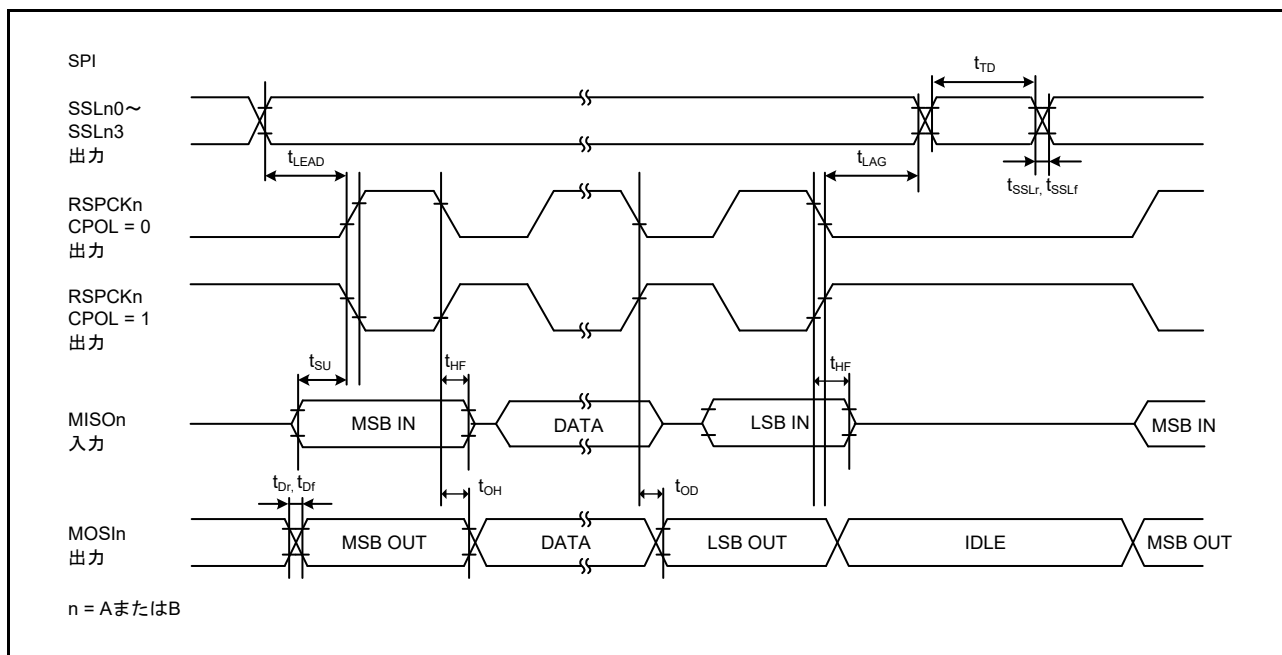
図 60.53 CPHA = 0 で、PCLKA/2 にピットレートが設定されている場合におけるマスタの SPI タイミング
