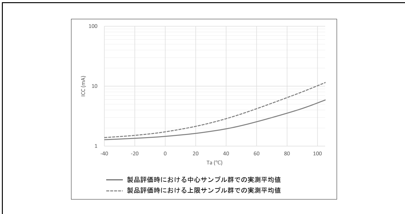
図 60.2 ソフトウェアスタンバイモード時の温度依存性 (参考データ)
