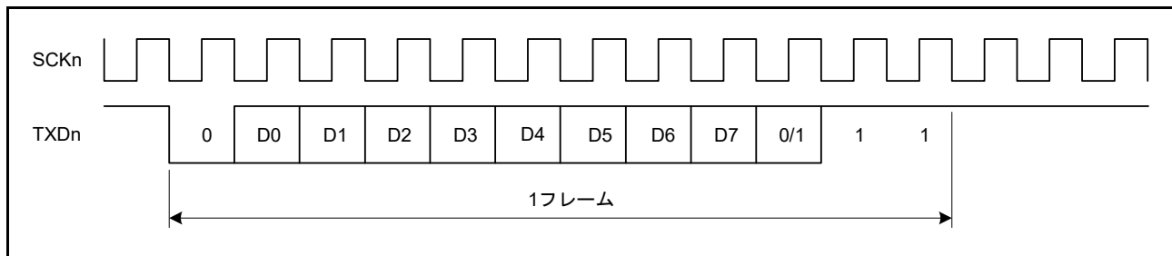
図 34.4 出力クロックと送信データの位相関係（調歩同期モード：SMR.CHR = 0、PE = 1、MP = 0、STOP = 1）
