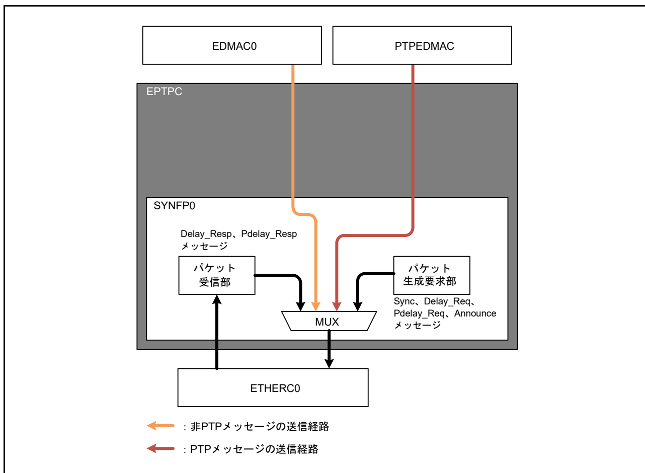
図 30.30 送信メッセージのアービトレーション
