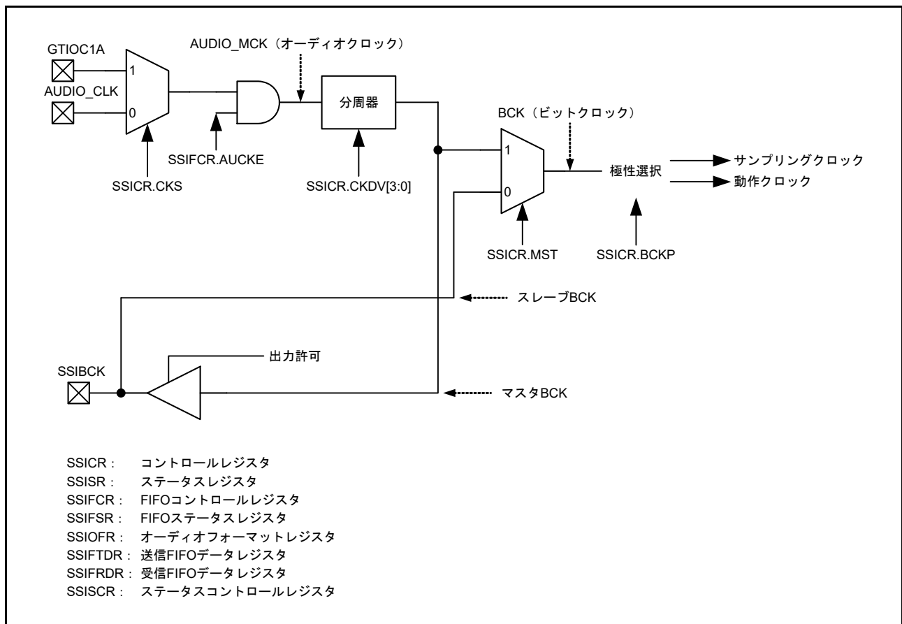
図 41.4 SSIE クロック構成
