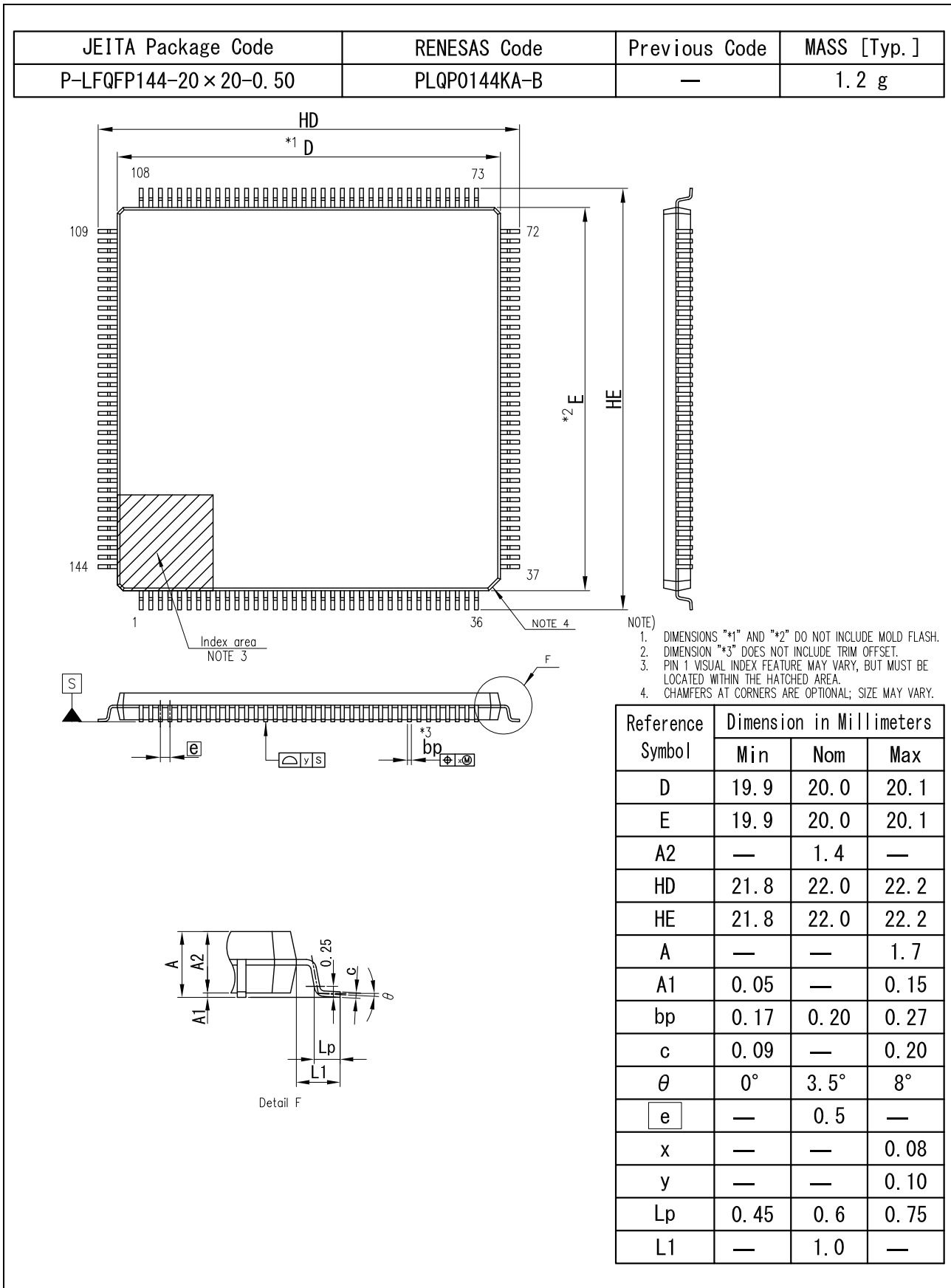
図 2.4 144-pin LQFP
