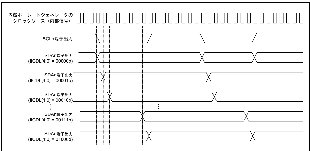
図 34.62 SDA 出力遅延のタイミング
