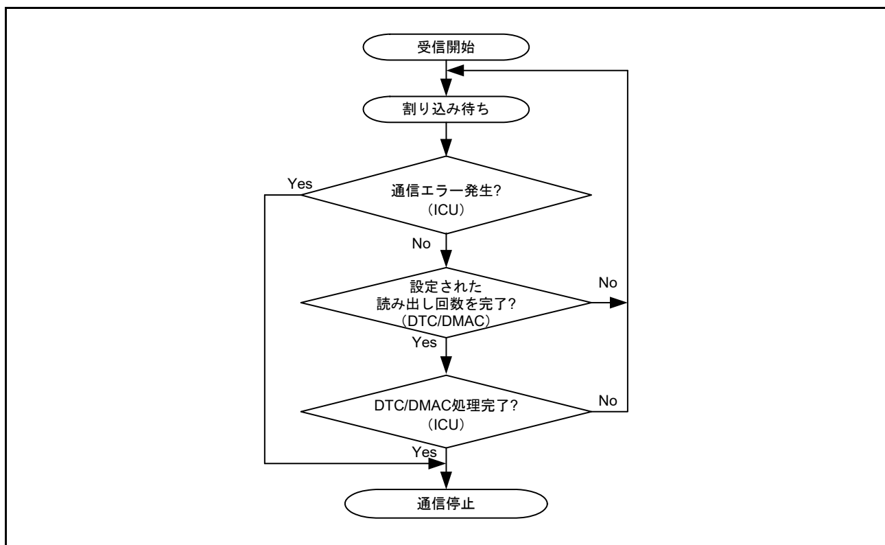
図 41.55 受信手順
