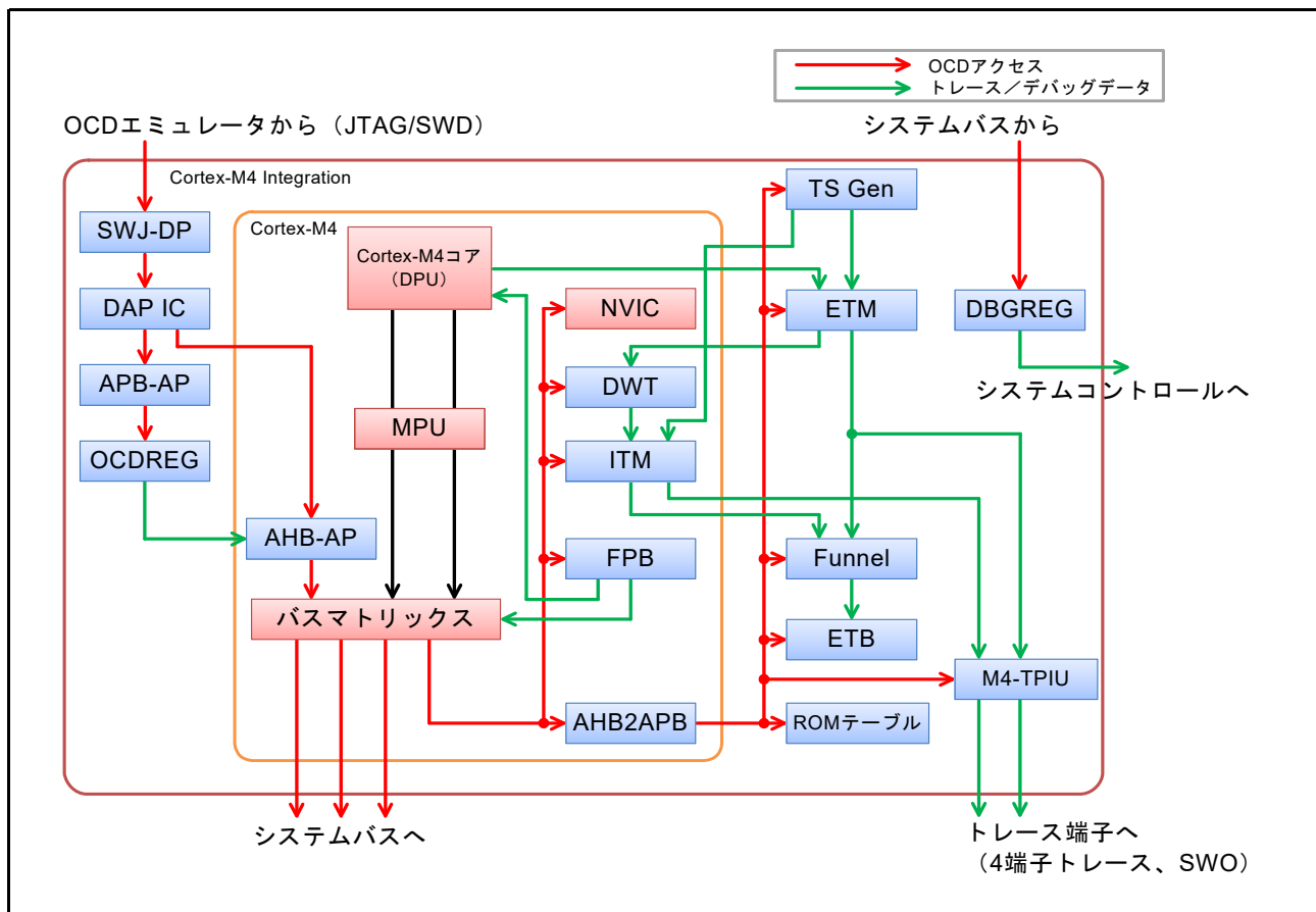
図 2.1 Cortex-M4 CPU ブロック図
