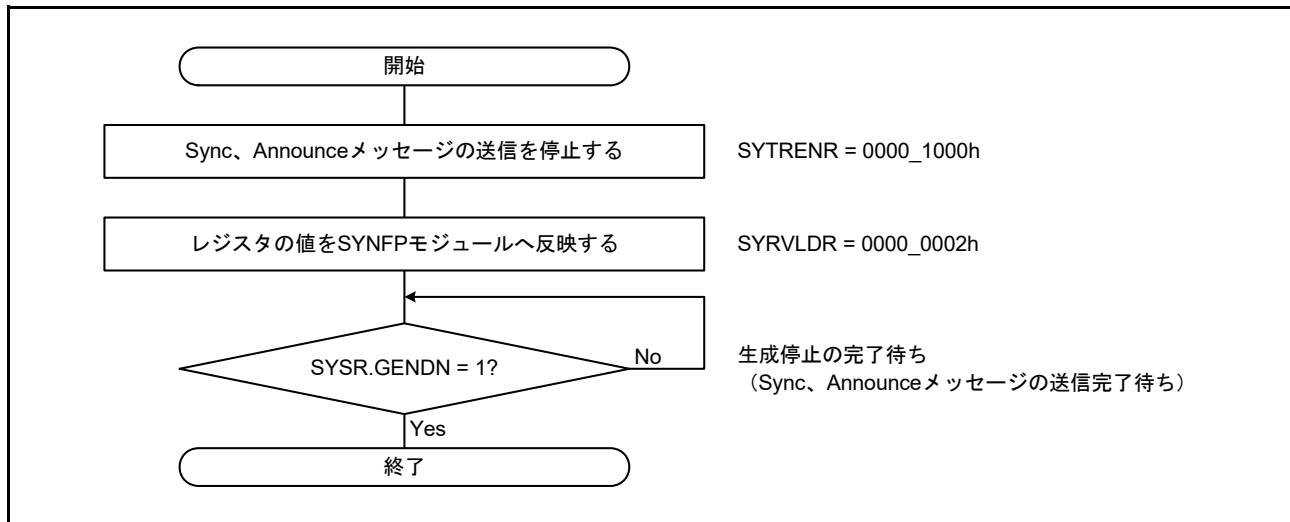
図 30.17 P2P マスタ動作の停止手順
