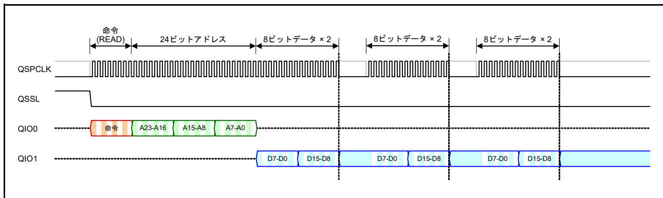
図 39.31 SPI バスサイクル拡張を使用した連続データのリード動作
