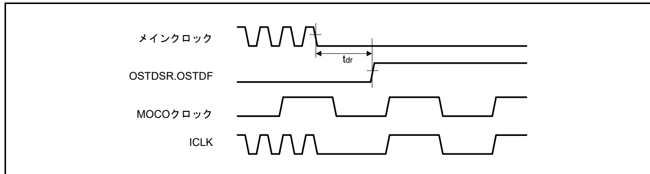
図 60.96 発振停止検出タイミング
