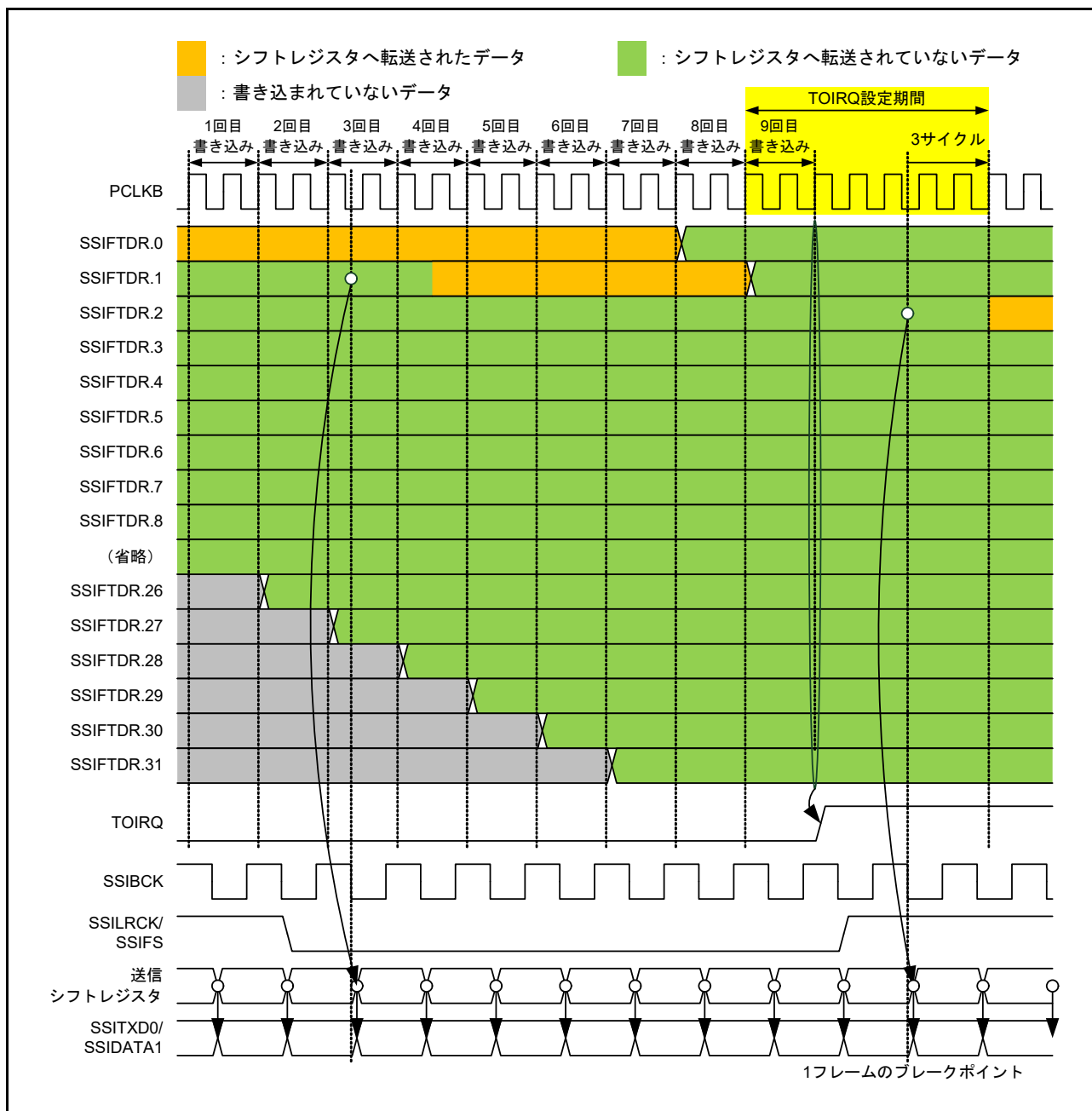
図 41.18 TOIRQ 設定タイミング
