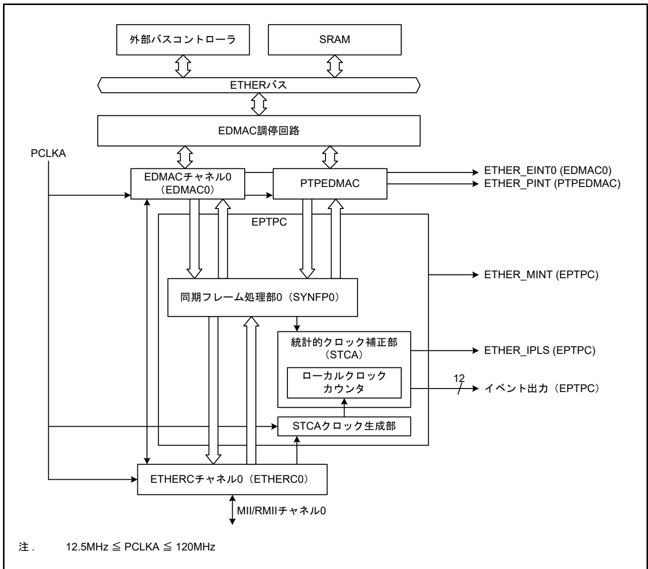
図 30.1 EPTPC の構成
