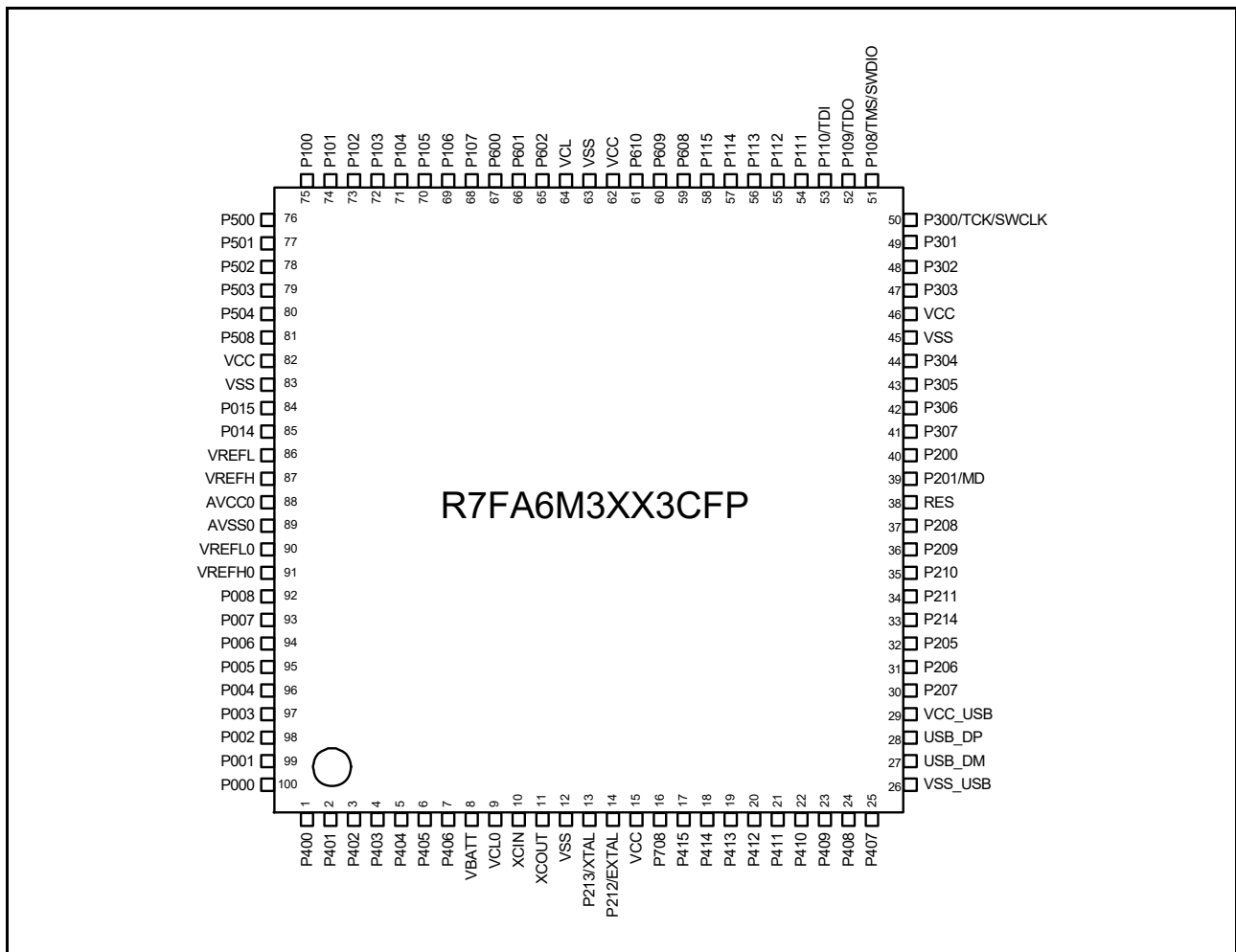
図 1.7 100-pin LQFP のピン配置図 (上面図)
