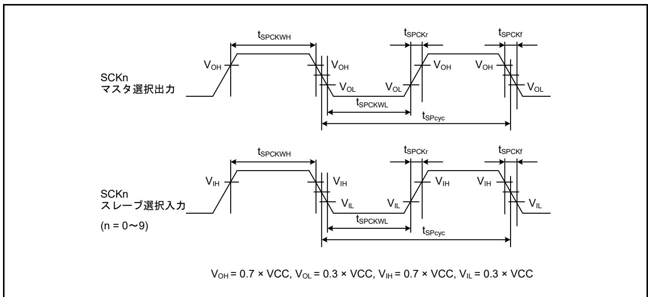
図 60.45 SCI簡易SPIモードクロックタイミング
