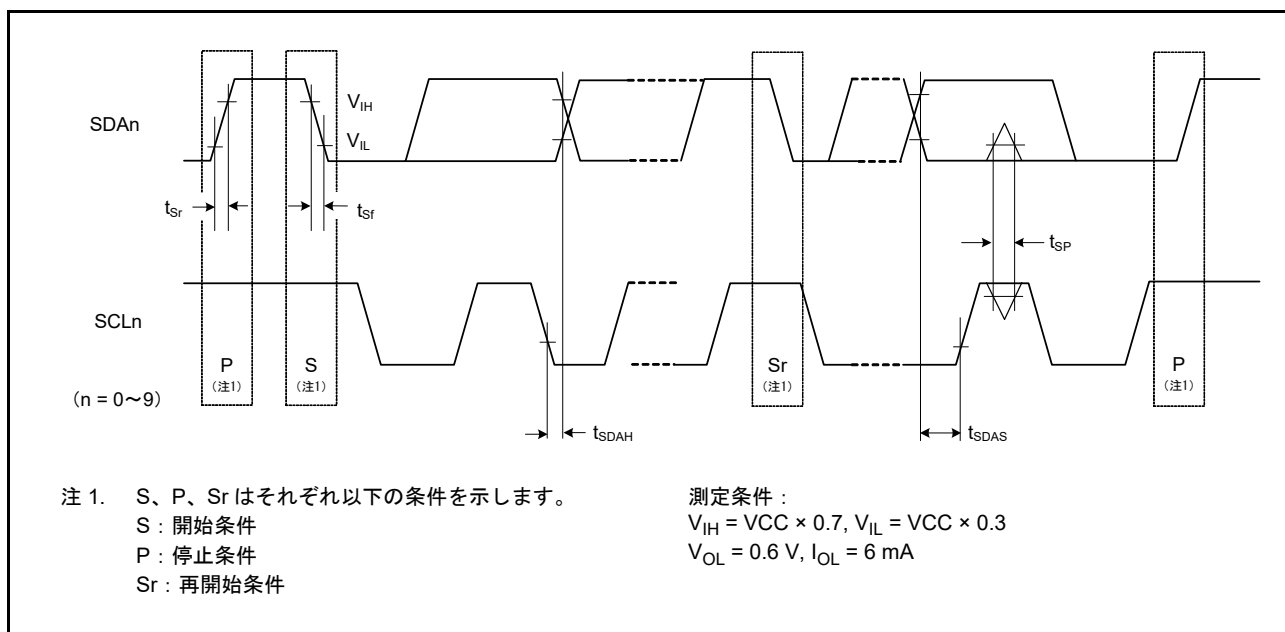
図 60.50 SCI 簡易 IIC モードタイミング
