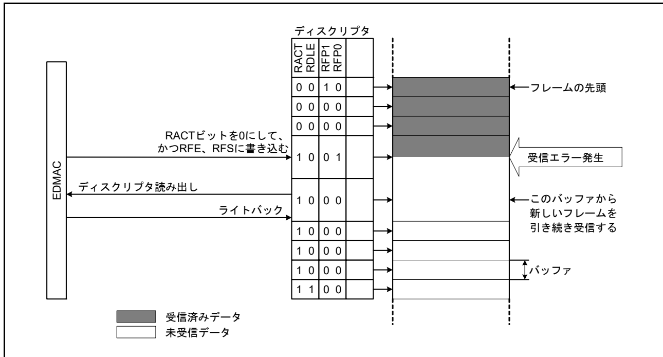
図 31.8 受信エラー発生後の EDMAC 動作
