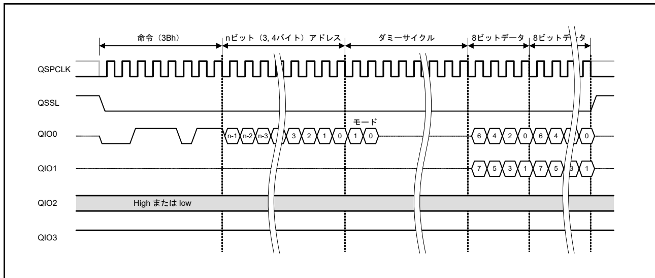
図 39.18 ファストリード Dual 出力バスサイクル
