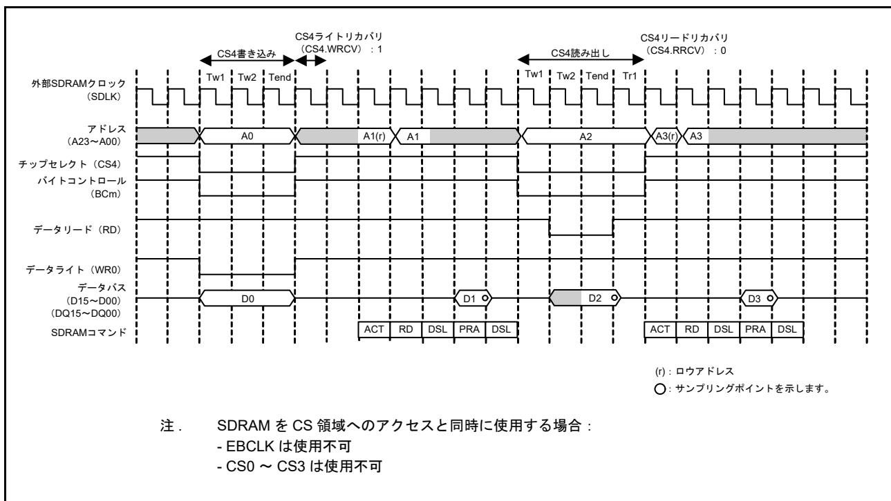
図 15.42 SDRAM アクセス時のリカバリタイミングの例
