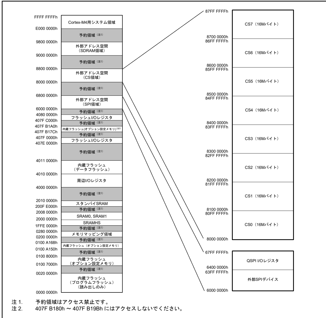
図 4.2 外部アドレス空間と CS 領域の対応
