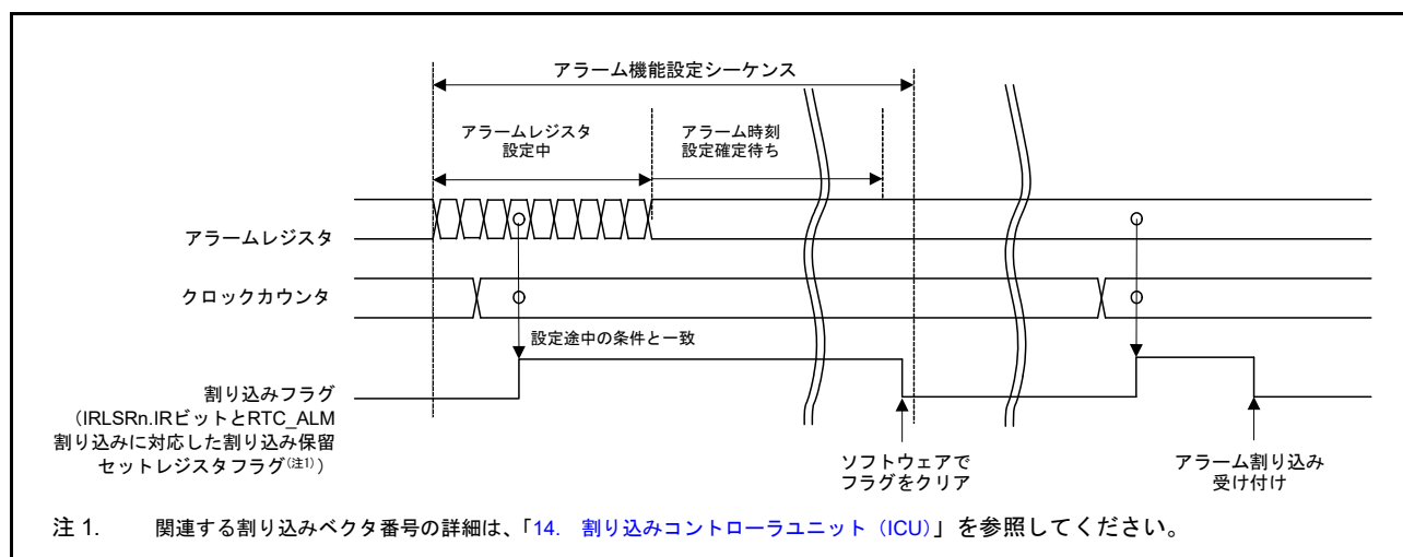
図 26.11 アラーム割り込み (RTC_ALM) のタイミング図
