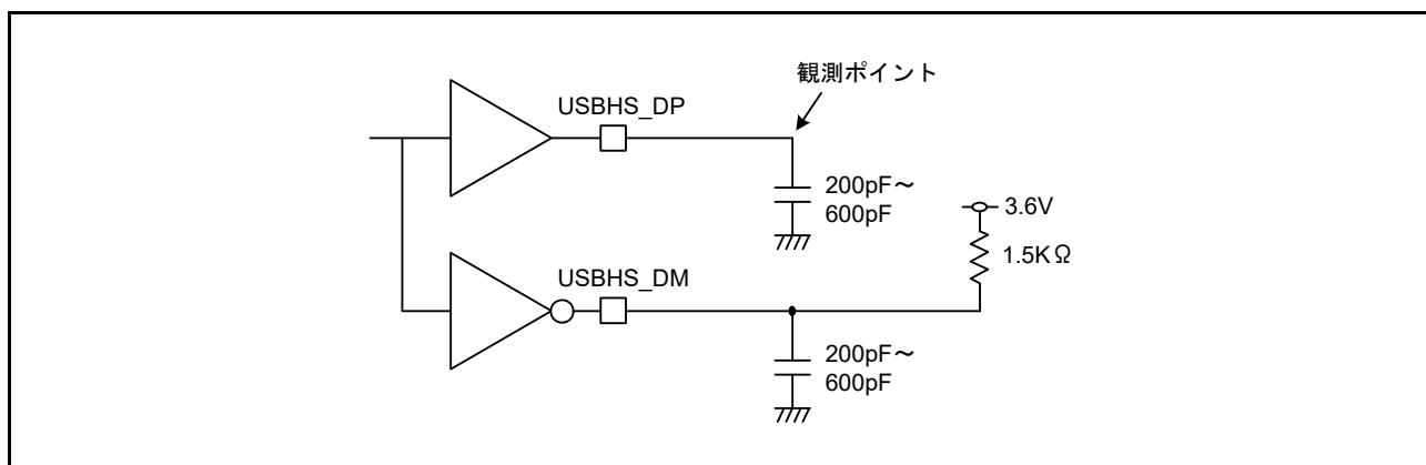
図 60.84 ロースピードモードにおける測定回路
