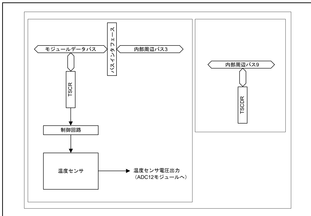
図 49.1 温度センサのブロック図
