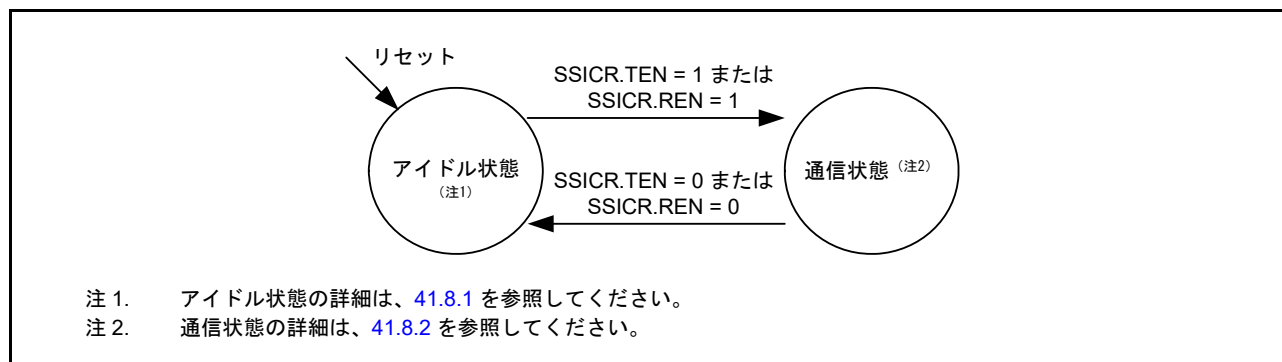
図 41.43 SSIE の状態遷移
