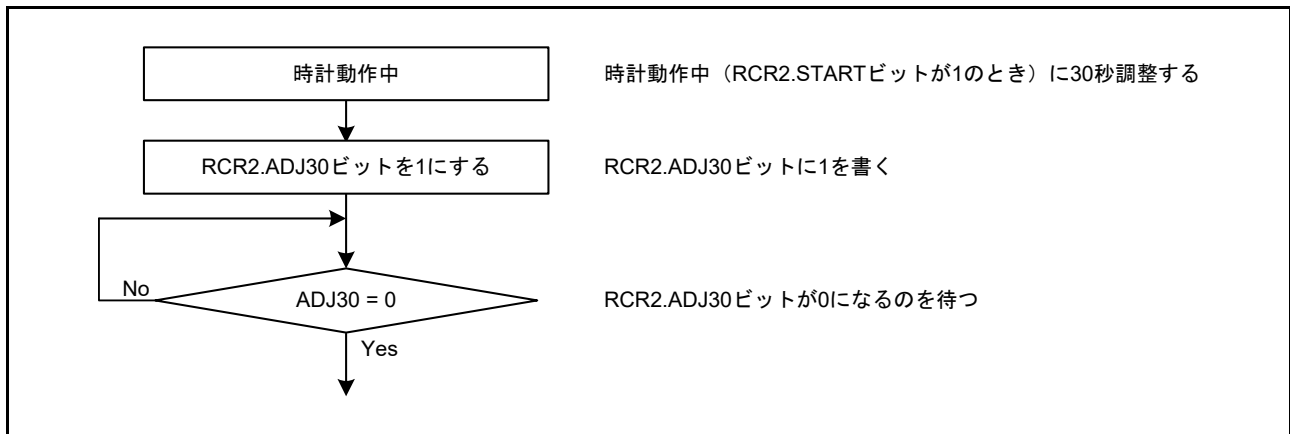
図 26.5 30 秒調整
