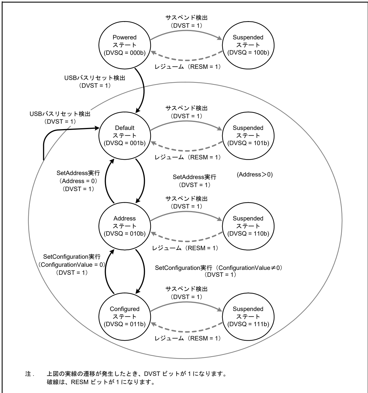
図 32.14 デバイスステートの遷移
