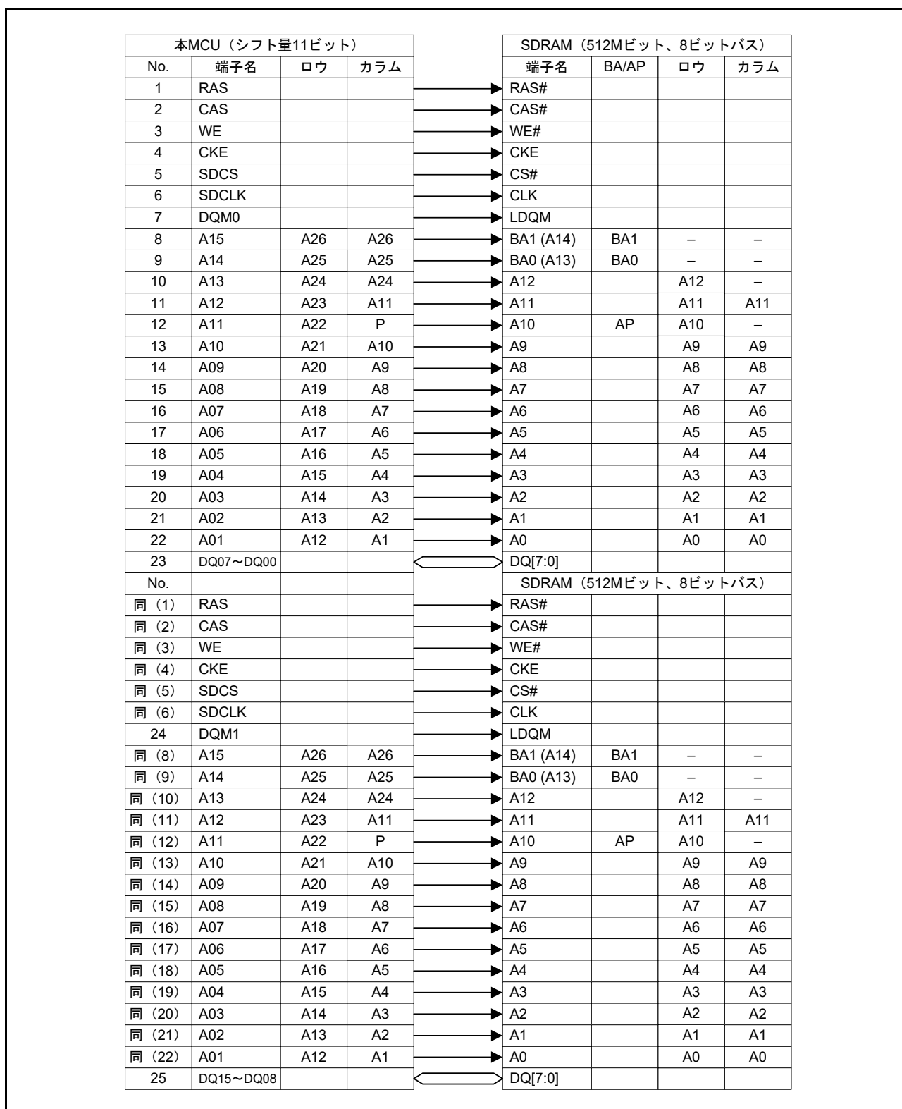
図 15.70 SDRAM 接続例 (512M ビット品 × 2 個、8 ビットバス)
