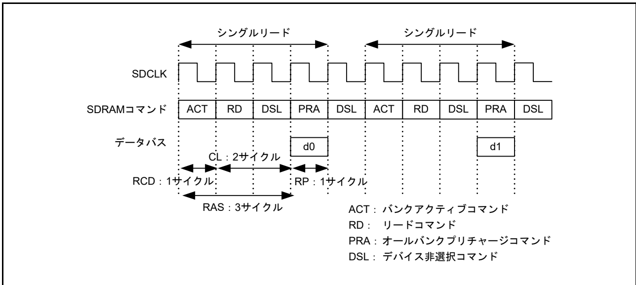
図 15.57 シングルリードタイミング例 (4)
