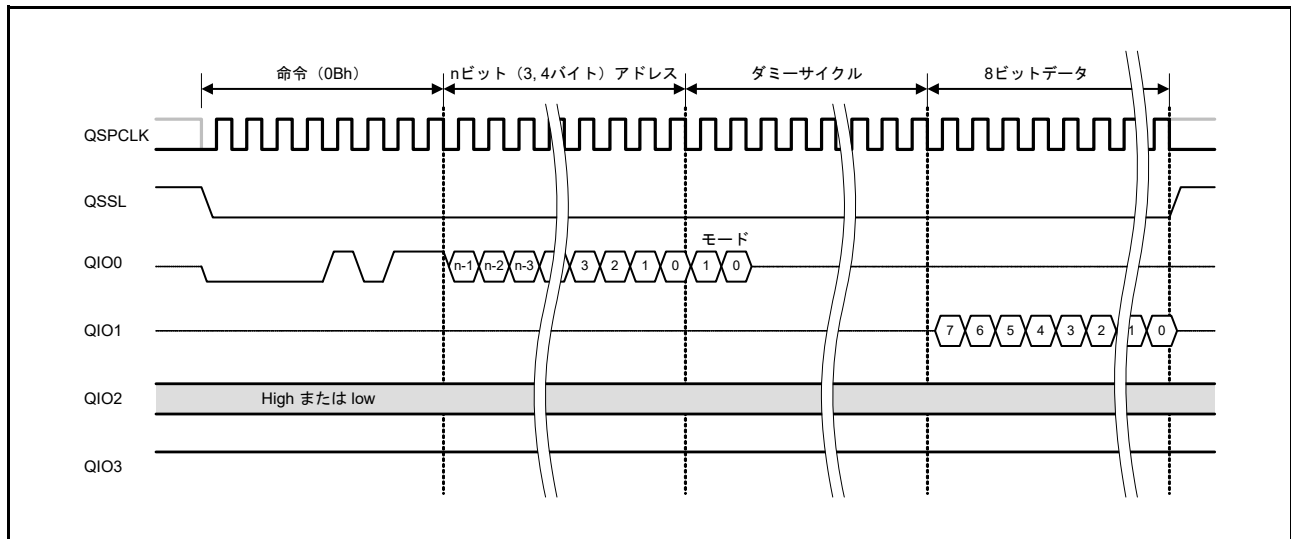
図 39.16 ファストリードバスサイクル
