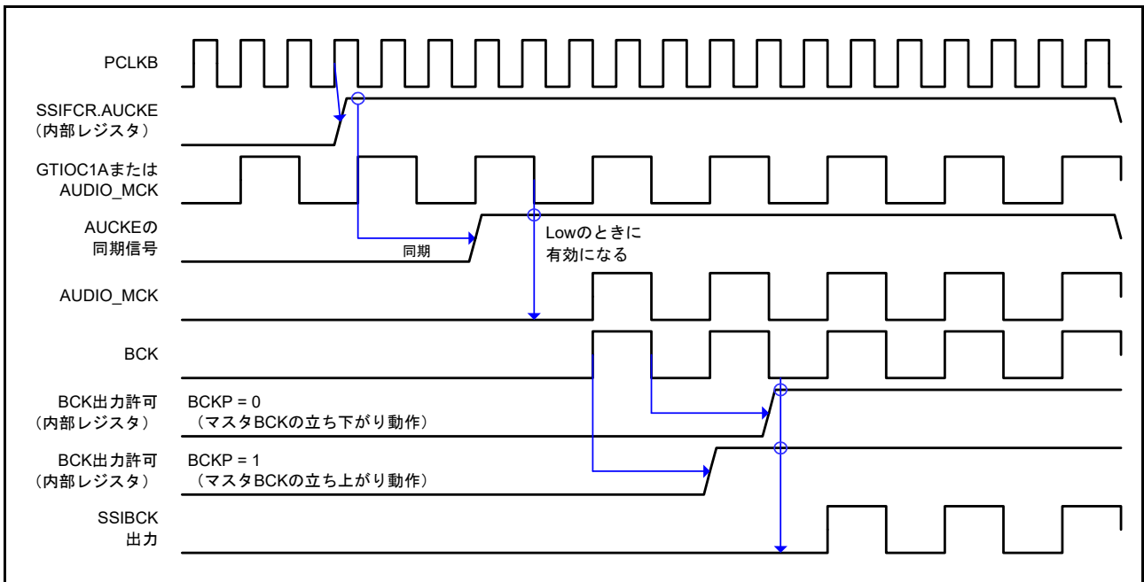
図 41.26 システムリセットからマスタモード通信開始までの動作のタイミング図
