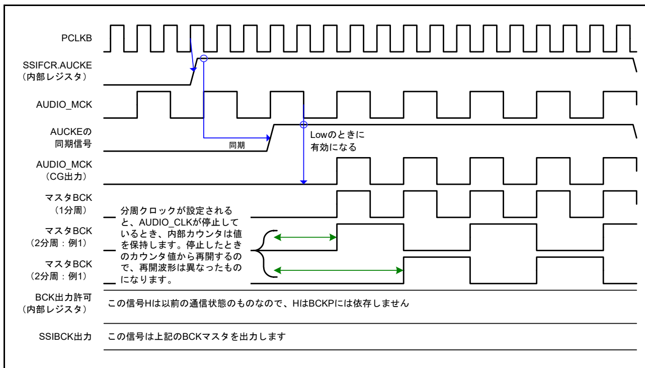
図 41.27 通信停止からマスタモード通信開始までの動作のタイミング図
