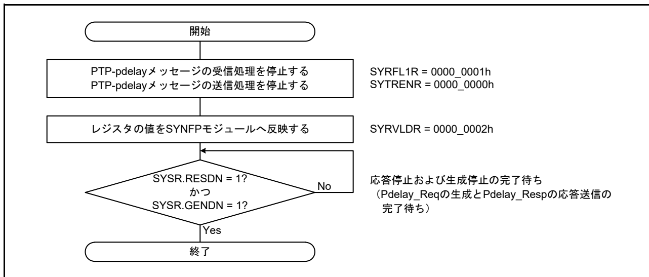
図 30.15 P2P 動作停止手順
