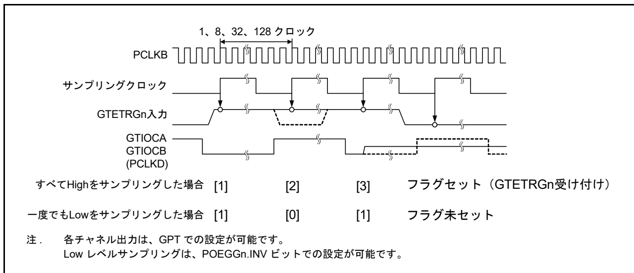
図 22.2 デジタルフィルタの動作例
