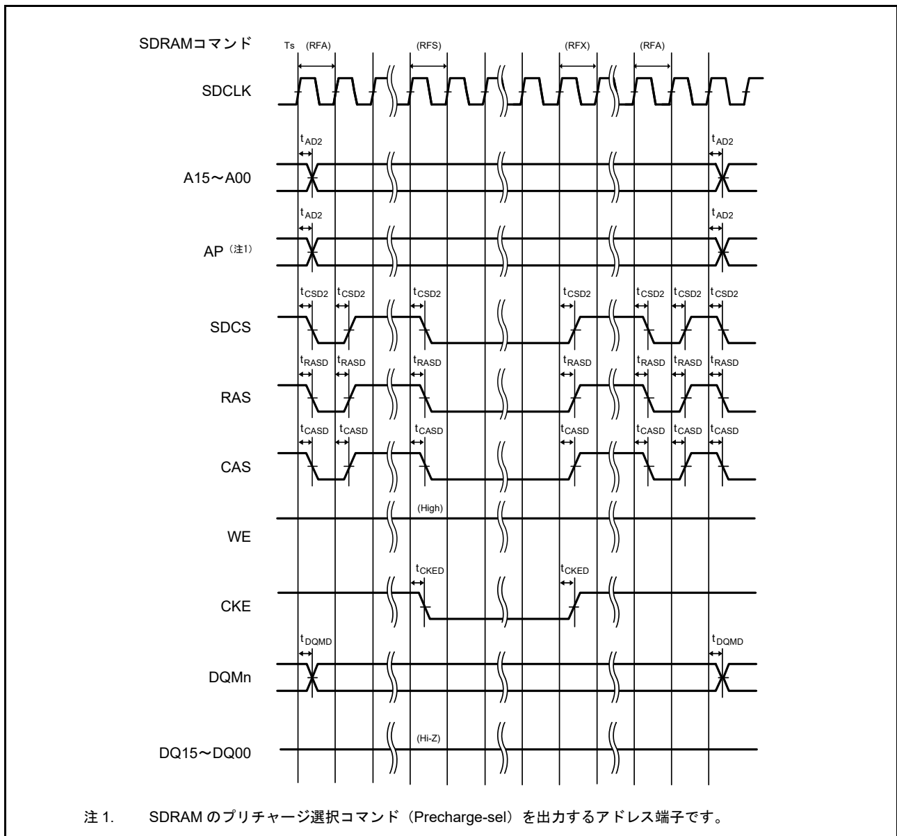
図 60.33 SDRAM セルフリフレッシュタイミング
