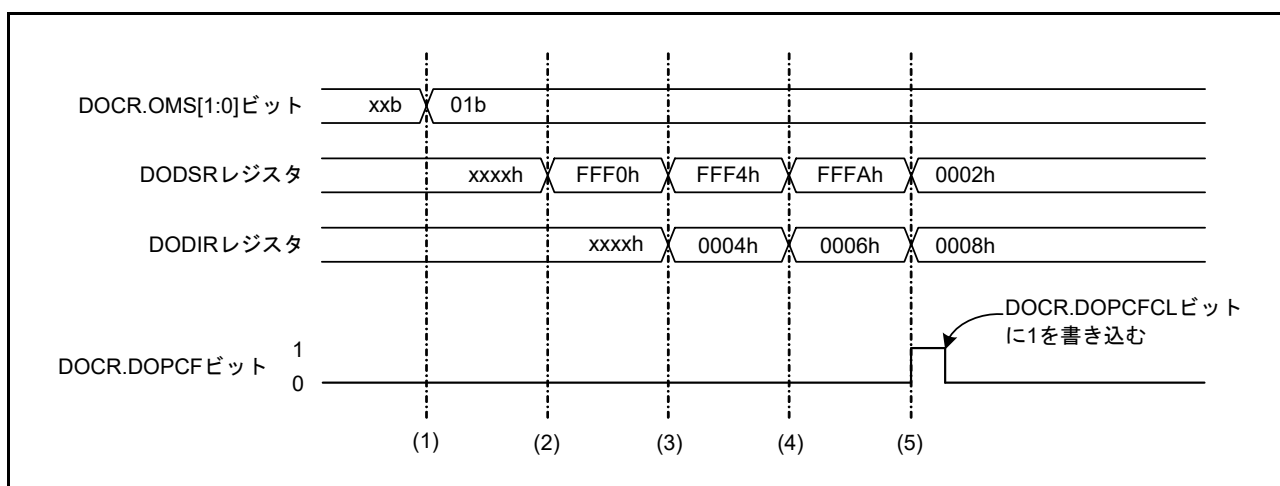
図 52.3 データ加算モードの動作例
