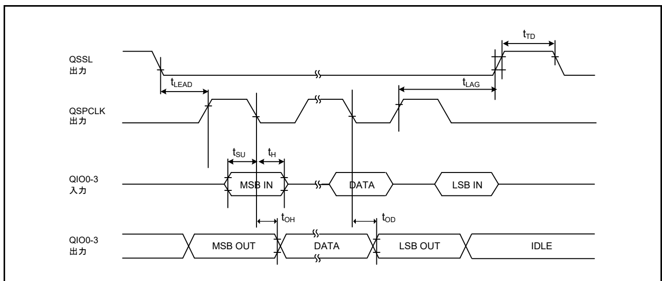
図 60.59 送受信タイミング
