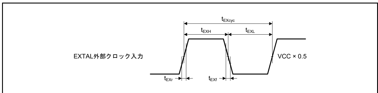
図 60.8 EXTAL 外部クロック入力タイミング
