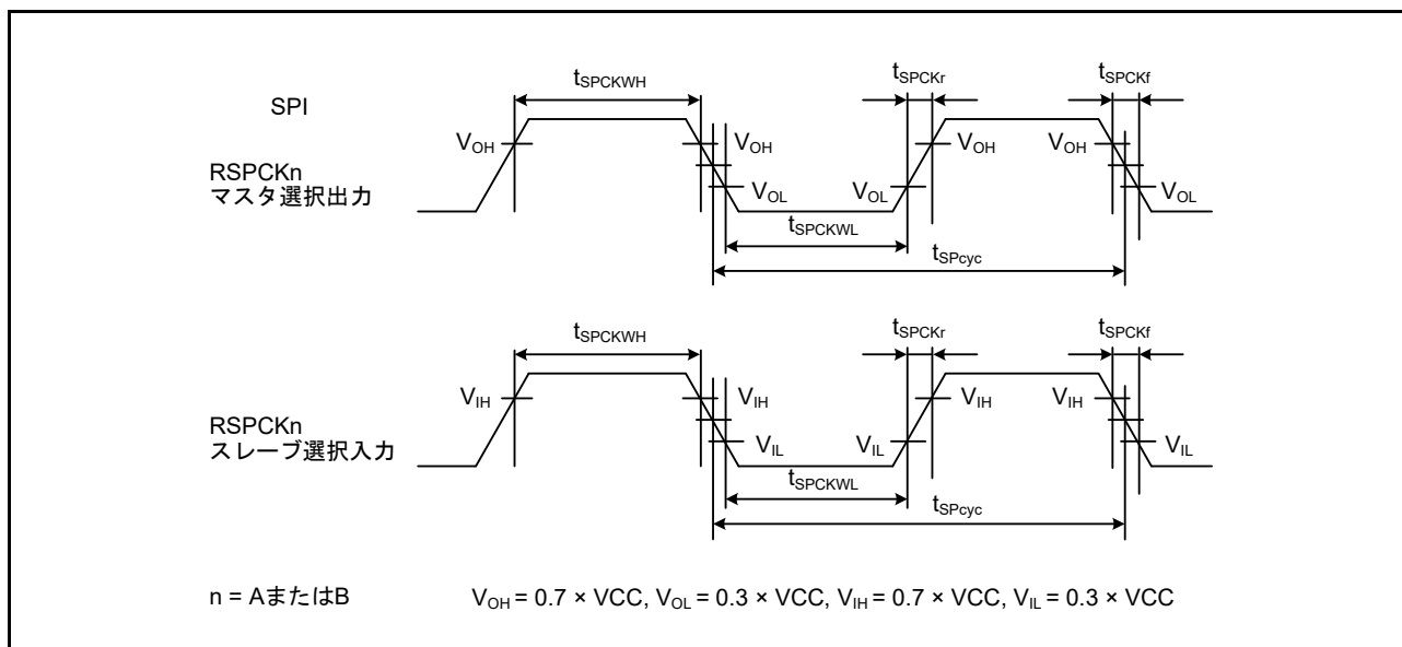
図 60.51 SPI クロックタイミング
