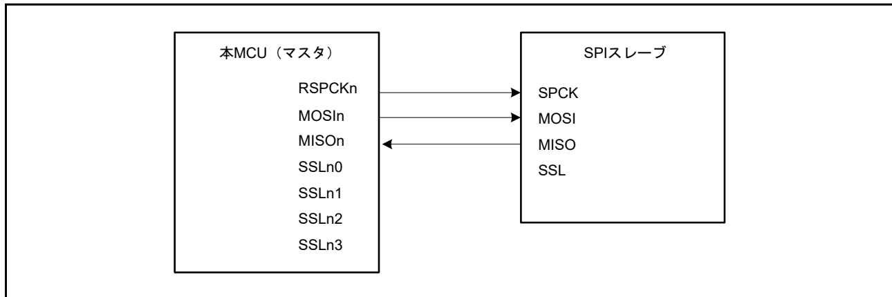
図 38.11 クロック同期式モードでのマスタ/スレーブの構成例 (MCU をマスタとして使用)
