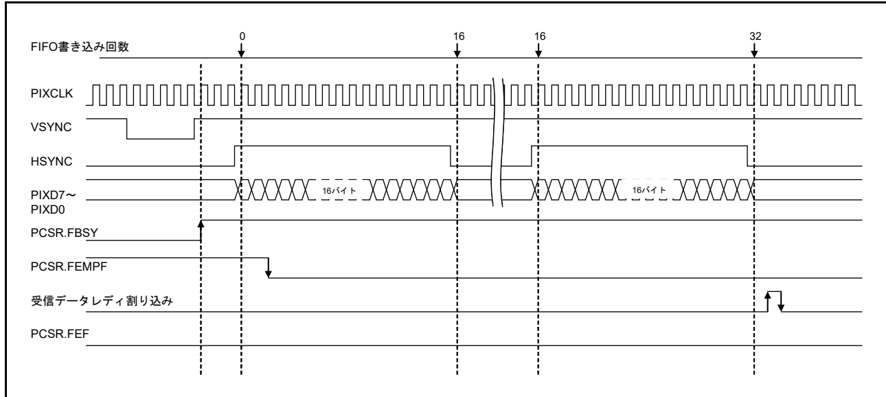
図 44.12 水平ブランキング期間中の動作例
