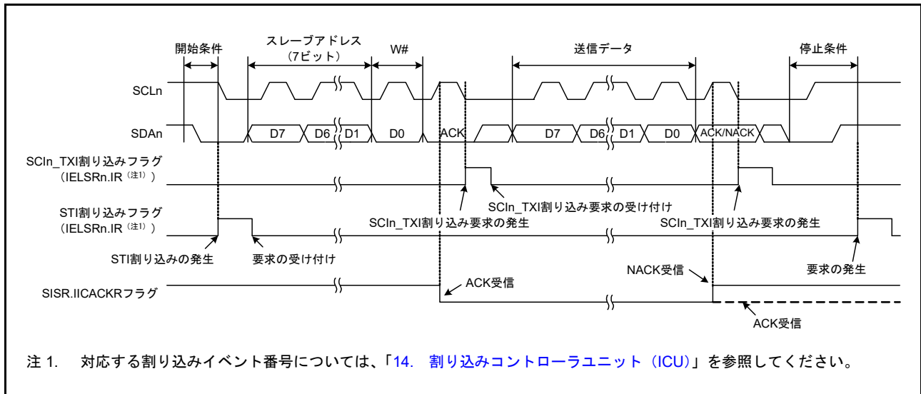
図 34.64 簡易 IIC モードにおけるマスタ送信の動作例 1 (7 ビットスレーブアドレス、送信割り込み、受信割り込み使用時)
