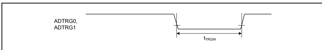
図 60.41 ADC12 トリガ入力タイミング
