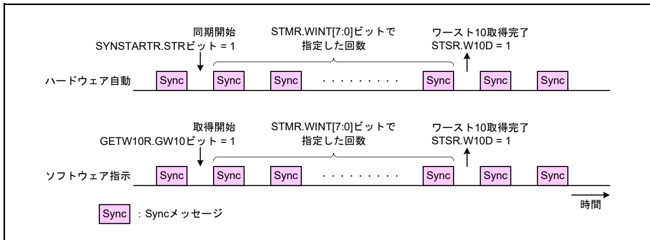
図 30.24 傾き差分値収集の概念
