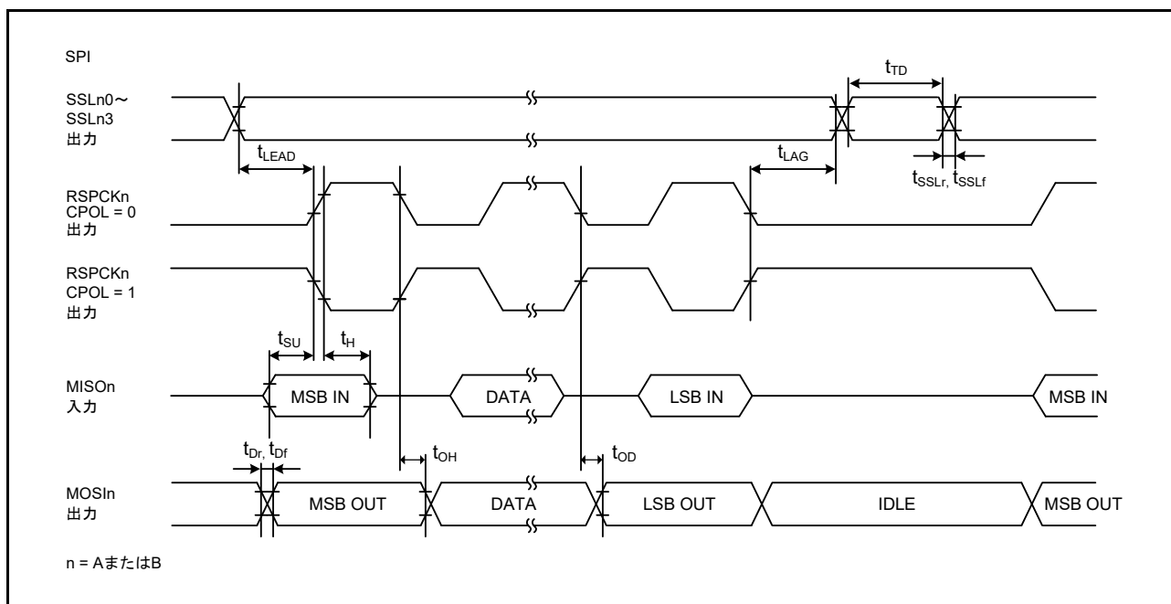
図 60.52 CPHA = 0 の場合におけるマスタの SPI タイミング
