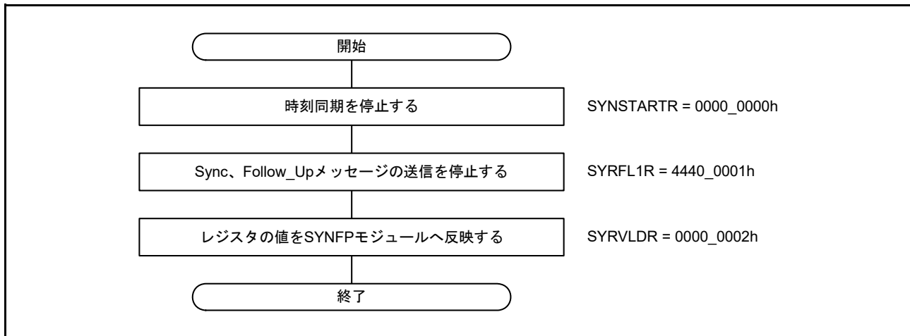
図 30.19 P2P スレーブ動作の停止手順
