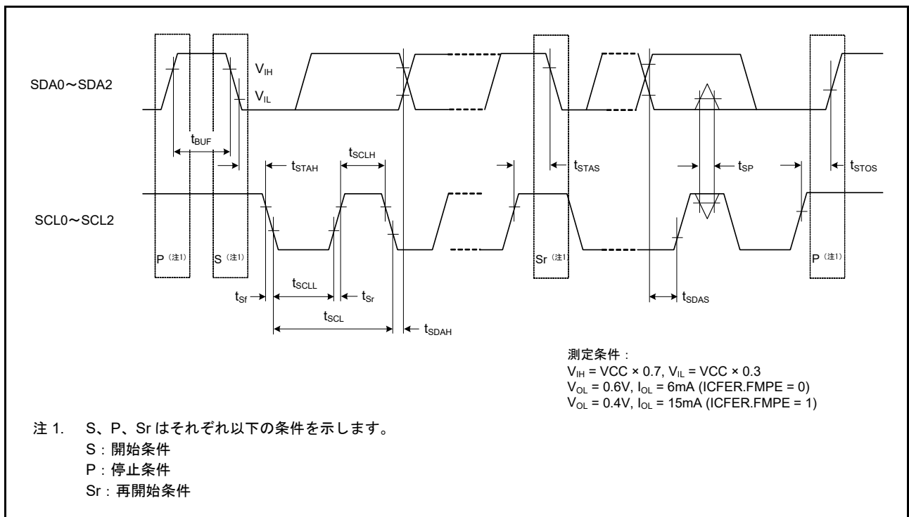
図 60.60 I2C バスインタフェース入出カタイミング
