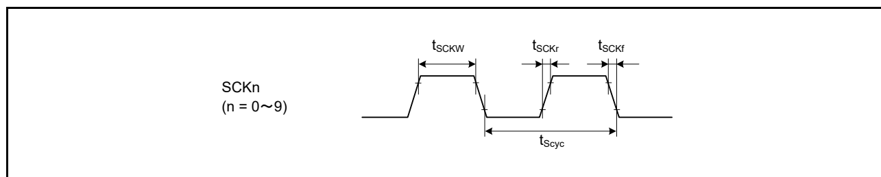
図 60.43 SCK クロック入出力タイミング
