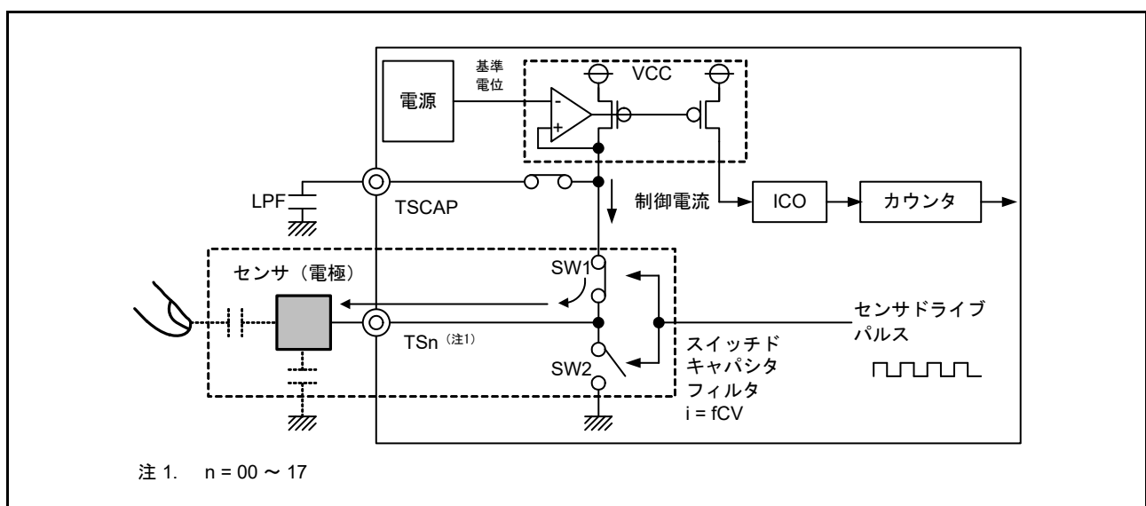
図 51.5 充電動作
