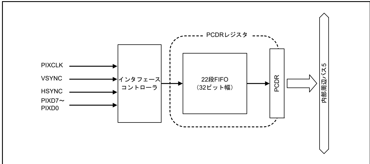
図 44.2 PCDR レジスタの構造図
