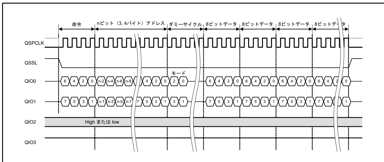
図 39.6 Dual-SPI プロトコル例 (ファストリード Dual I/O)
