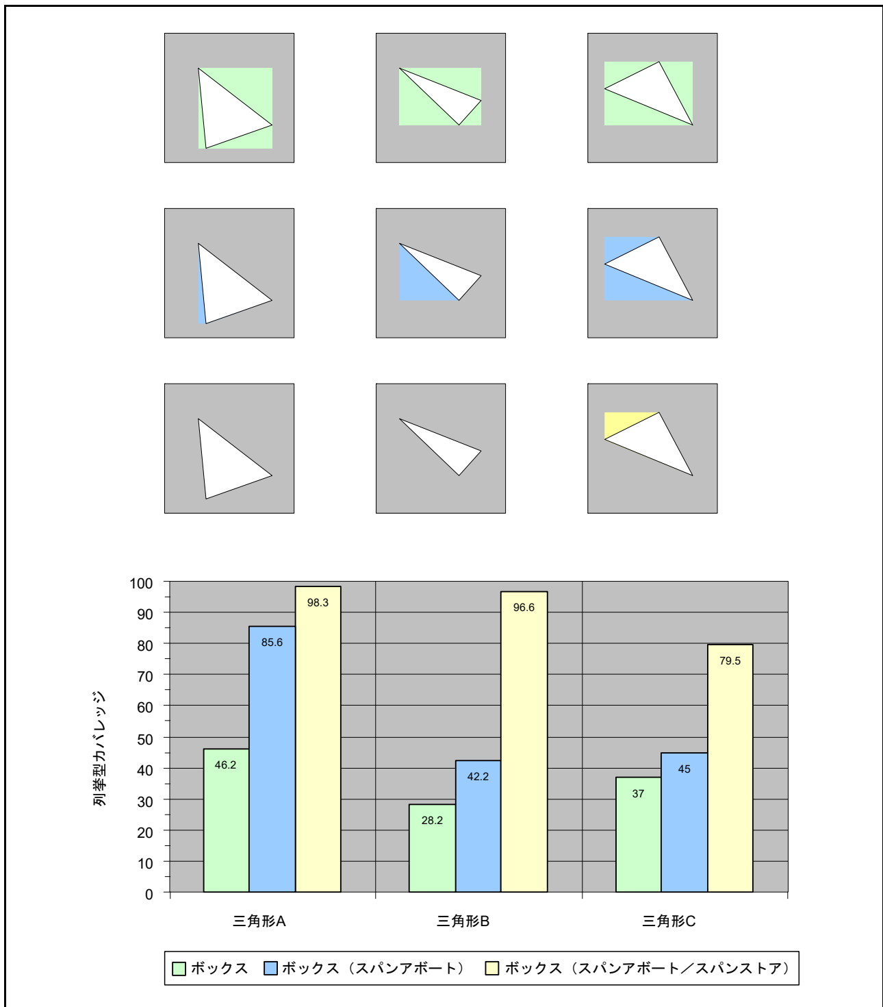
図 56.19 列挙型カバレッジ = {プリミティブのピクセル/バウンディングボックスのピクセル} の場合のスパンストアおよびスパニアポート最適化の効率
