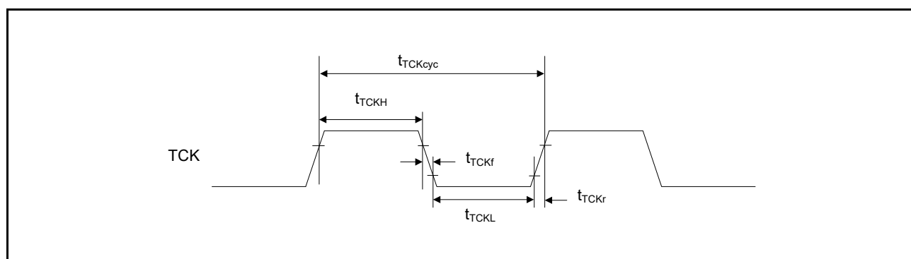
図 60.106 JTAG TCK タイミング
