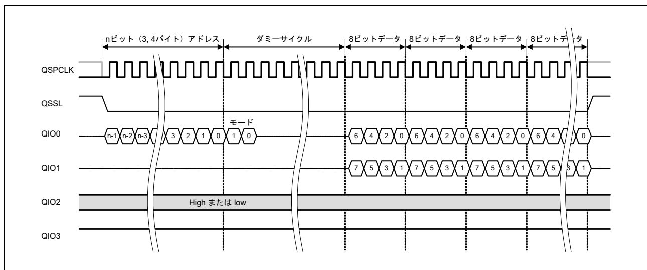
図 39.19 XIP モード時のファストリード Dual 出力バスサイクル
