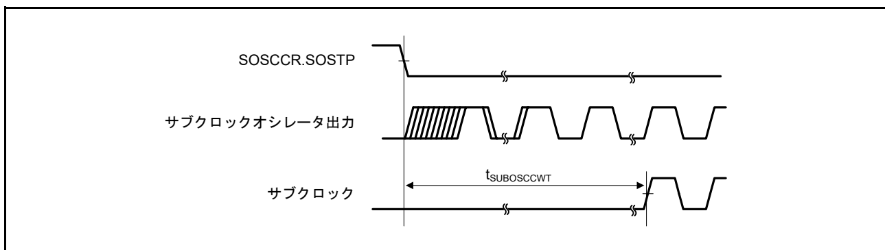
図 60.12 サブクロック発振開始タイミング
