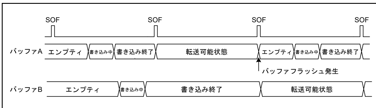
図 32.21 バッファフラッシュ動作例
