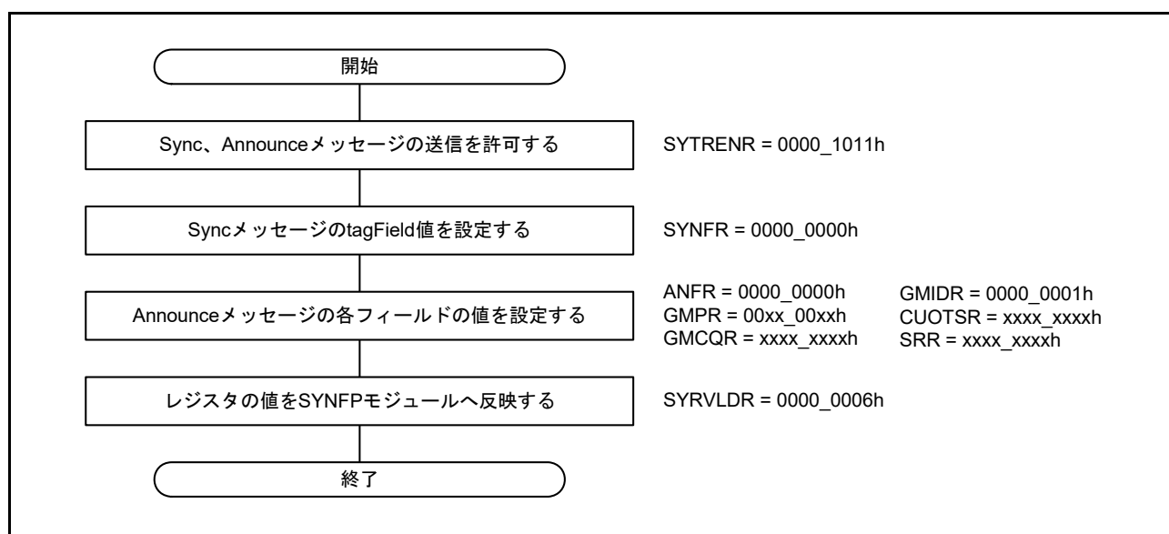
図 30.16 P2P マスタ動作の開始手順
