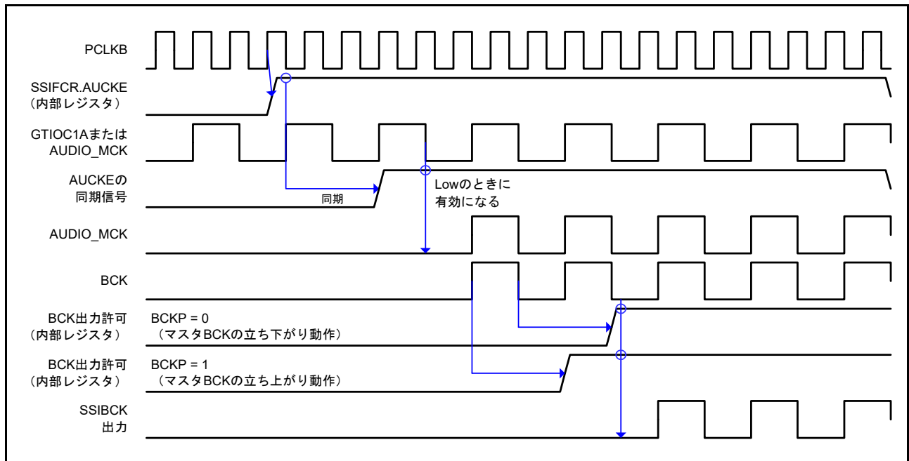
図 41.26 システムリセットからマスタモード通信開始までの動作のタイミング図
