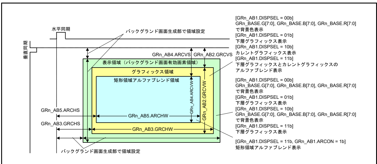
図 58.8 グラフィックディスプレイの選択
