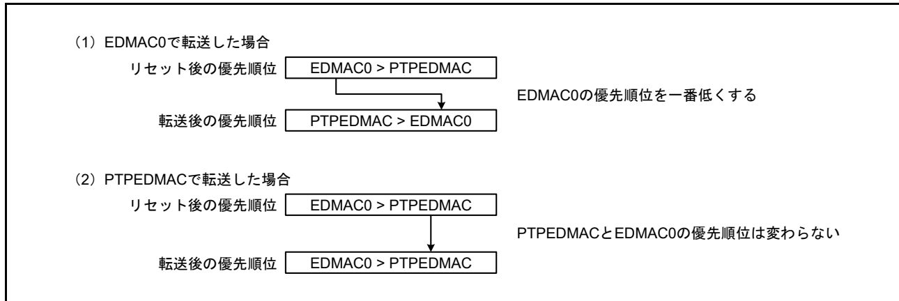
図 31.9 チャンネルの優先順位
