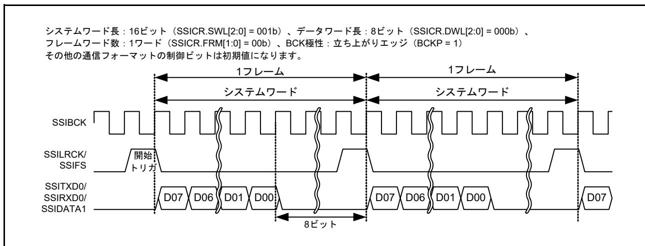
図 41.39 モノラルフォーマットでのショートフレーム (パディングあり、システムワード長 > データワード長)
