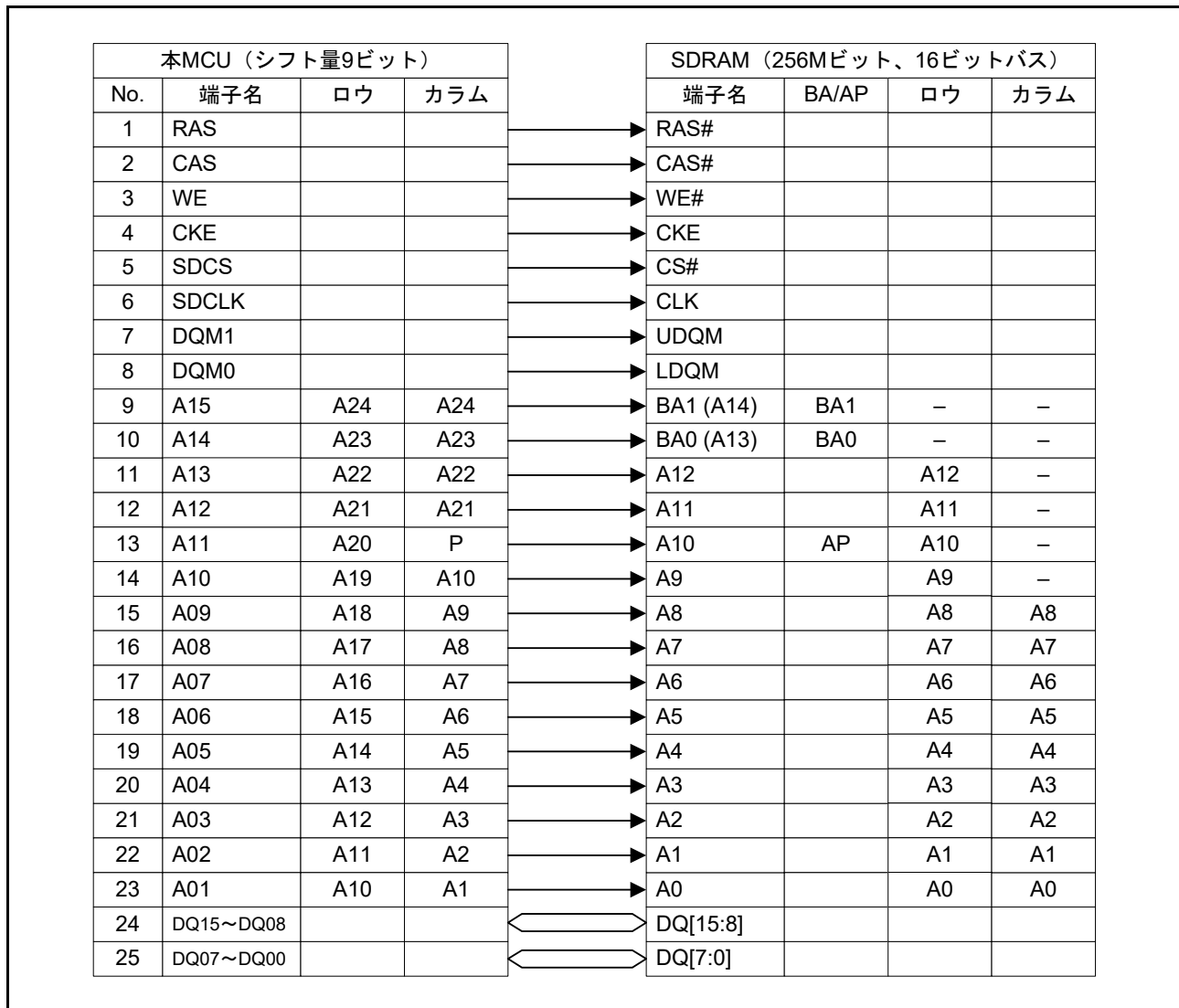
図 15.72 SDRAM 接続例 (256M ビット品 × 1 個、16 ビットバス)
