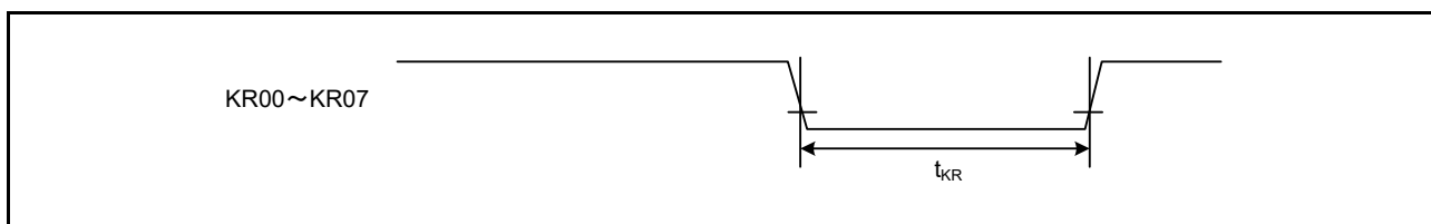
図 60.42 キー割り込み入力タイミング
