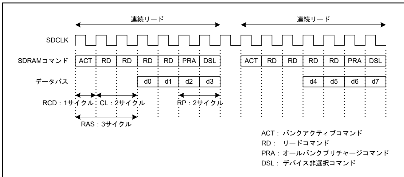
図 15.64 連続リードタイミング例 (1)
