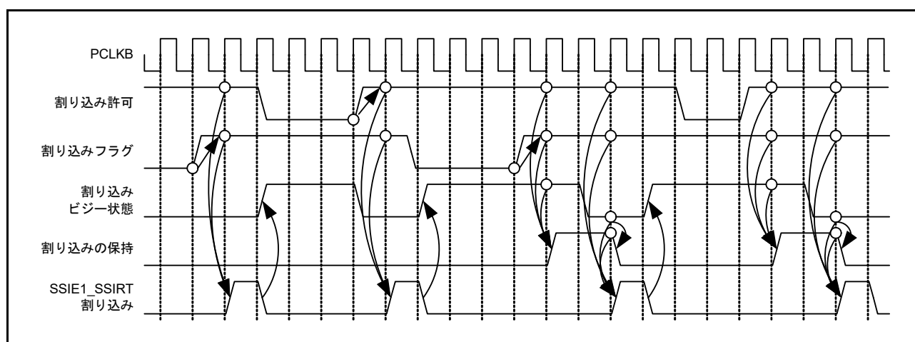
図 41.61 SSIE1_SSIRT 割り込みのタイミング図
