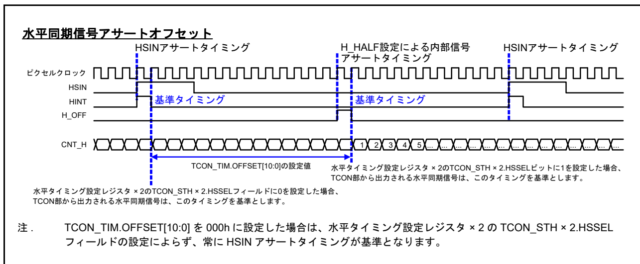
図 58.15 TCON における水平同期信号生成の基準タイミング
