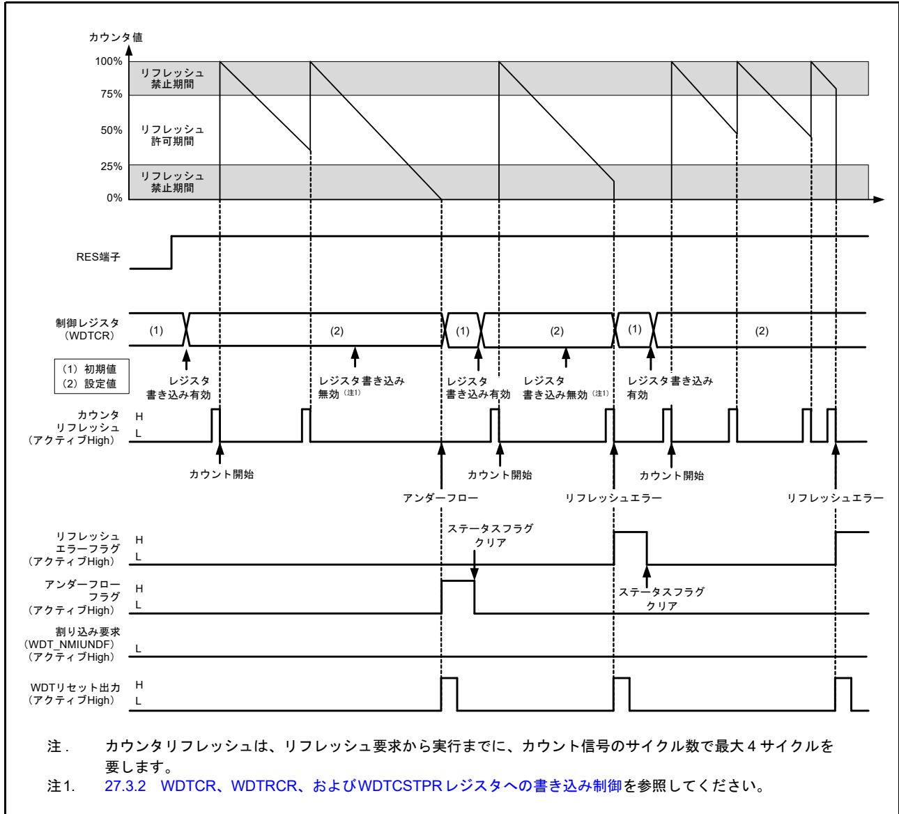
図 27.3 レジスタスタートモードでの動作例
