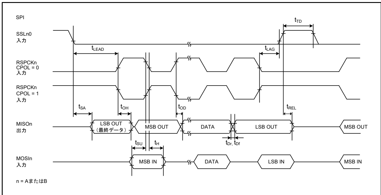
図 60.57 CPHA = 1 の場合におけるスレーブの SPI タイミング
