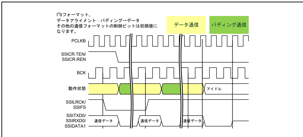
図 41.50 データ通信からの停止 (パディングビットあり)
