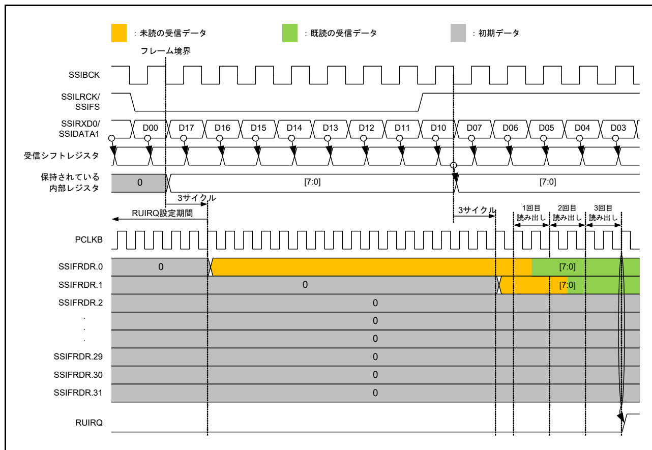
図 41.17 RUIRQ 設定タイミング
