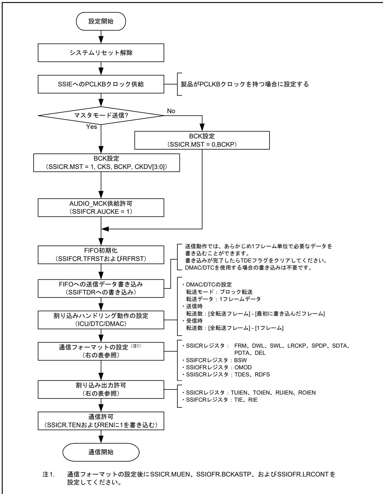
図 41.53 通信開始手順 (CPU 動作手順)
