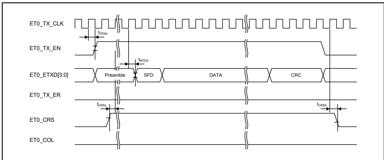
図 60.72 正常動作時の MII 送信タイミング
