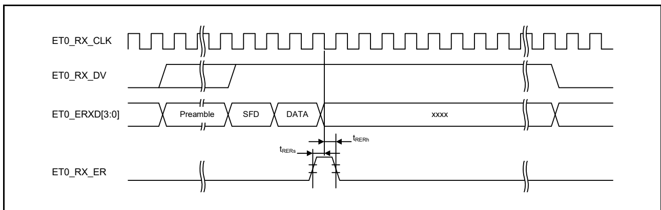
図 60.75 エラー発生時の MII 受信タイミング
