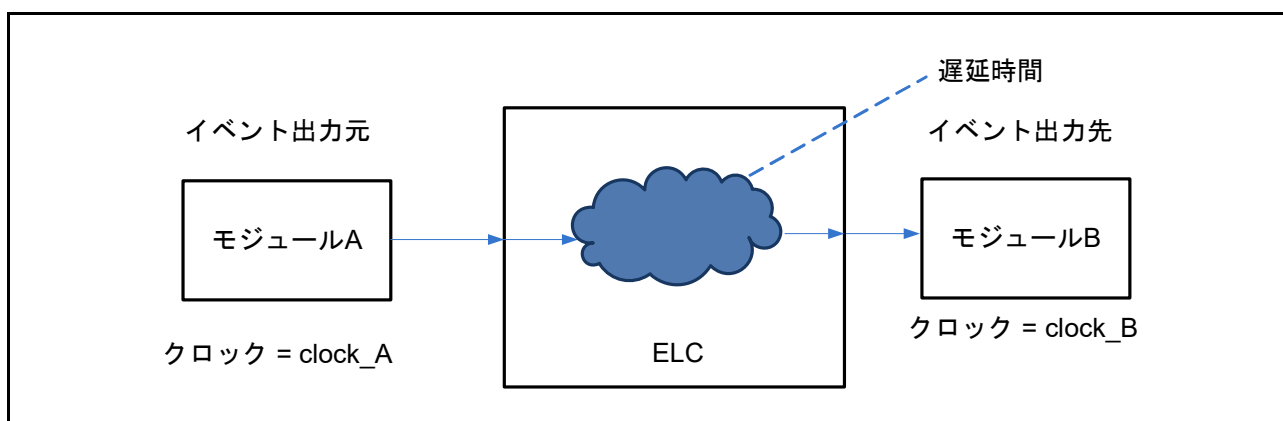
図 19.2 ELC 遅延時間
