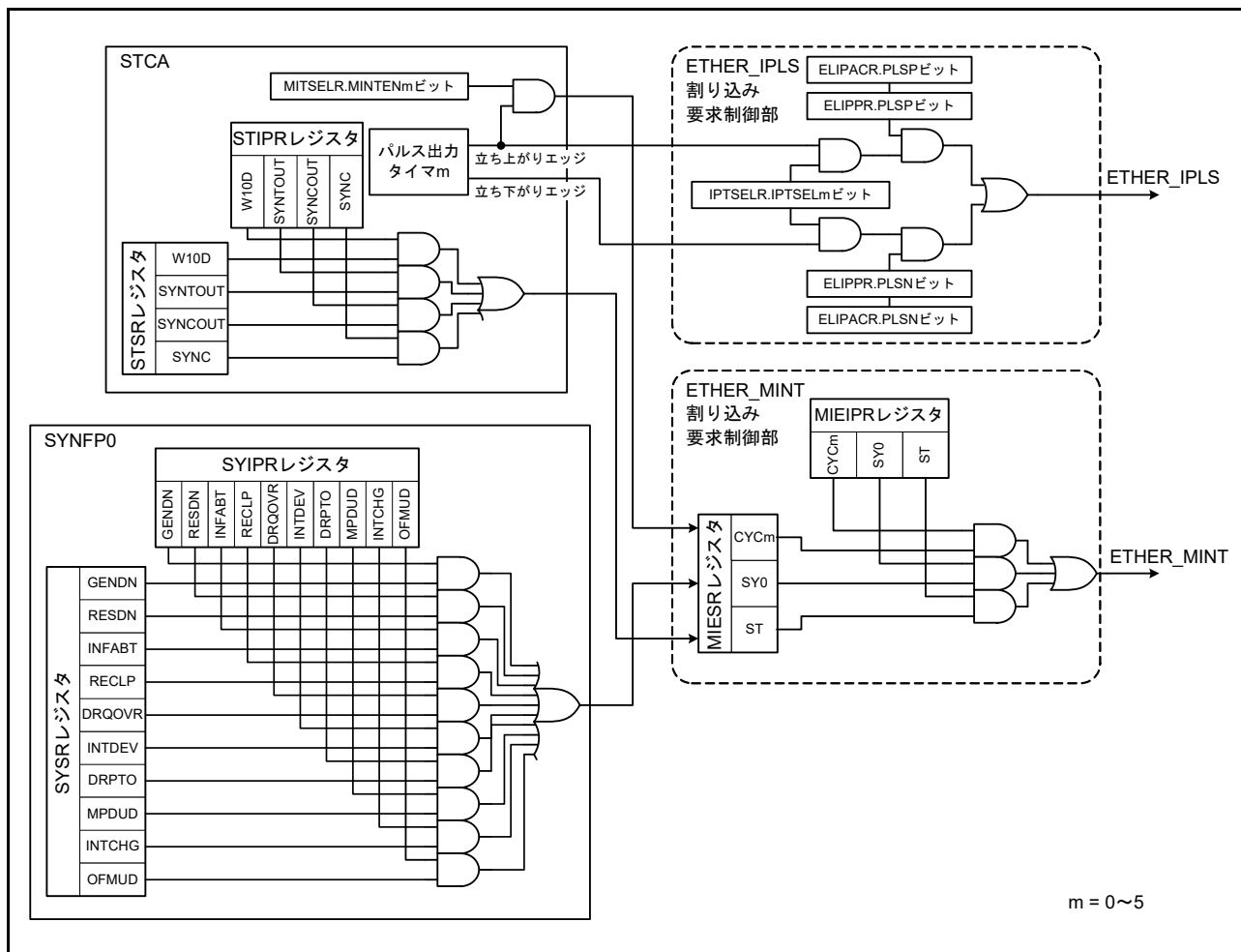
図 30.32 ETHER_MINT と ETHER_IPLS 割り込み要求
