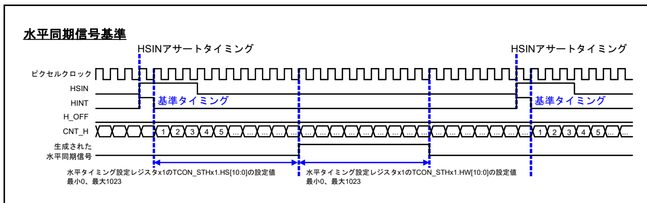
図 58.20 入力水平同期信号 (HSIN) に基づく信号生成
