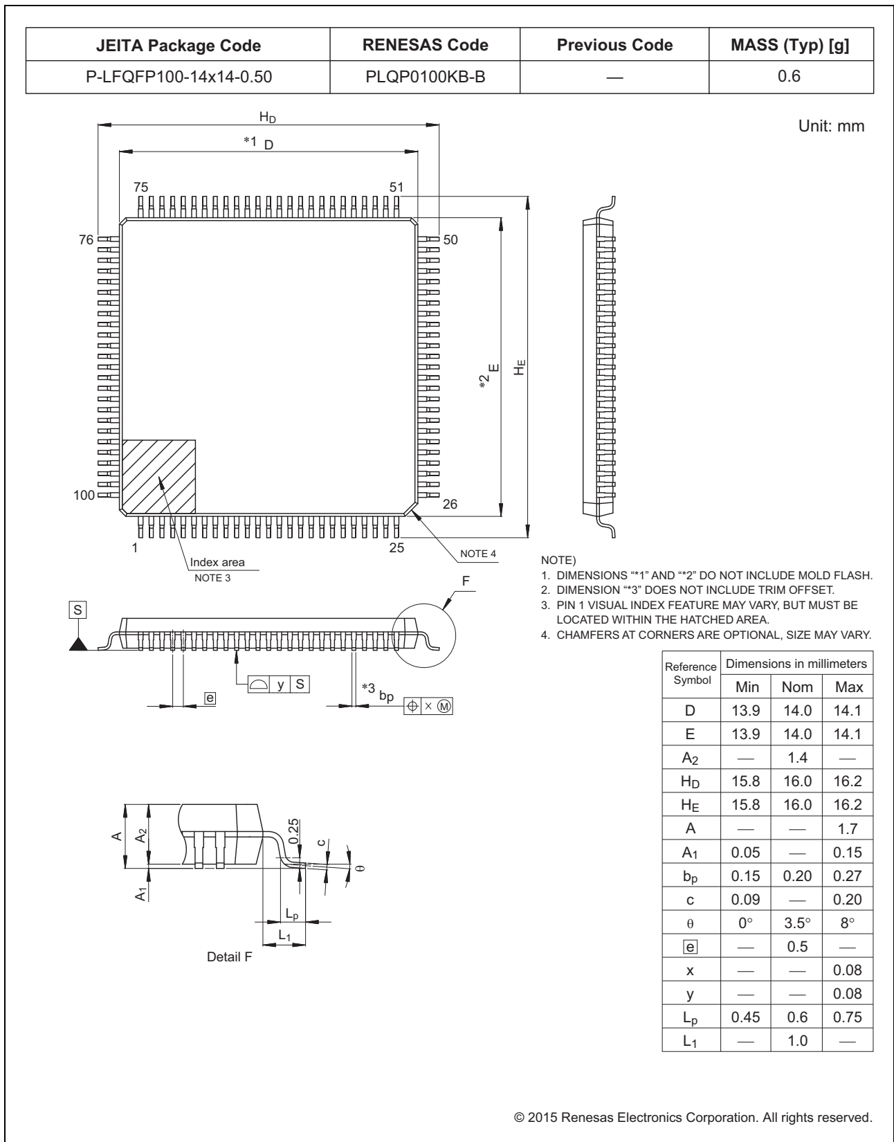
図 2.5 100-pin LQFP
