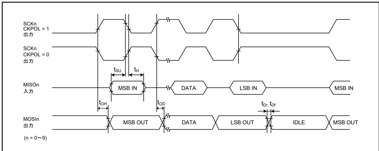
図 60.47 CKPH = 0 の場合におけるマスタの SCI 簡易 SPI モードタイミング
