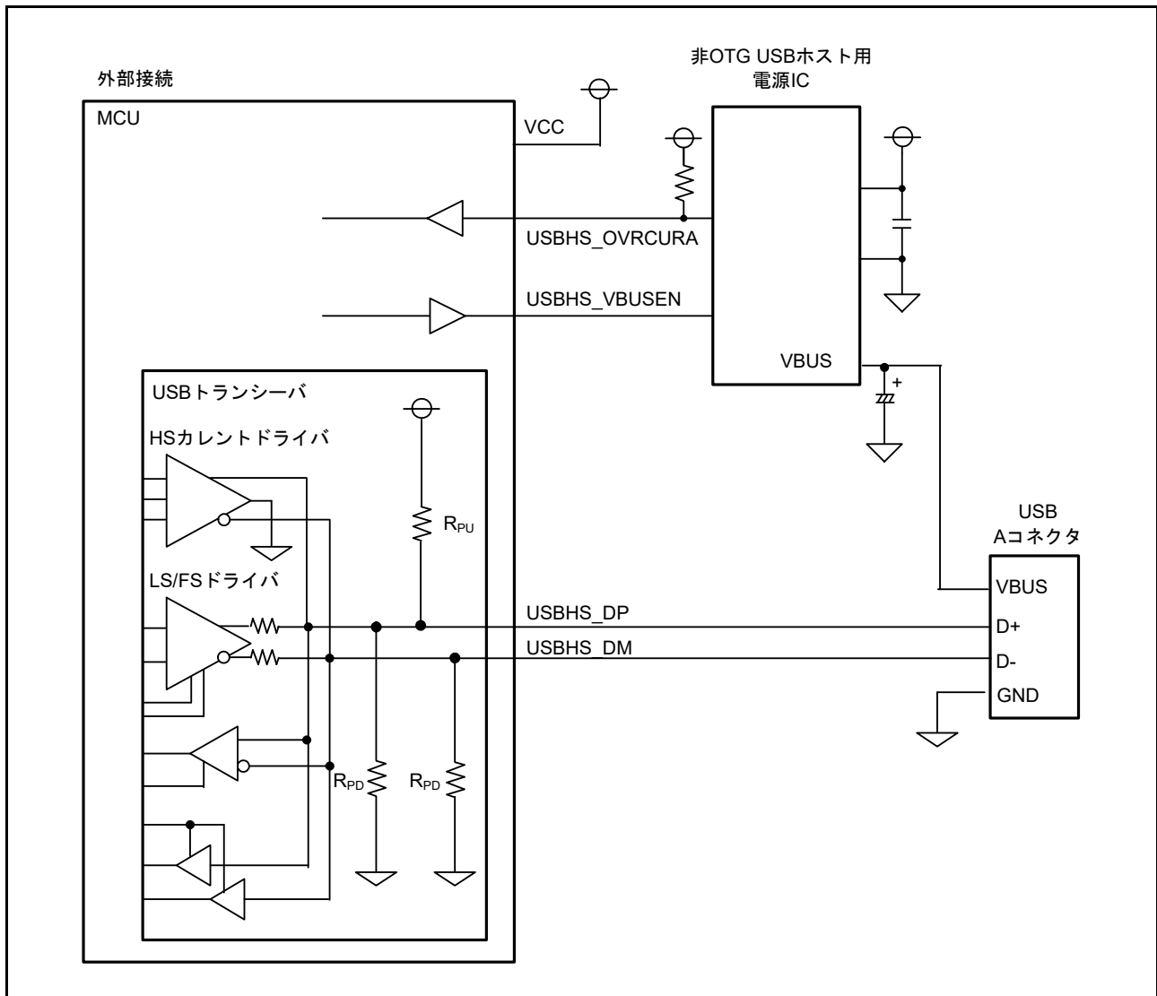
図 33.30 USB ホスト接続例
