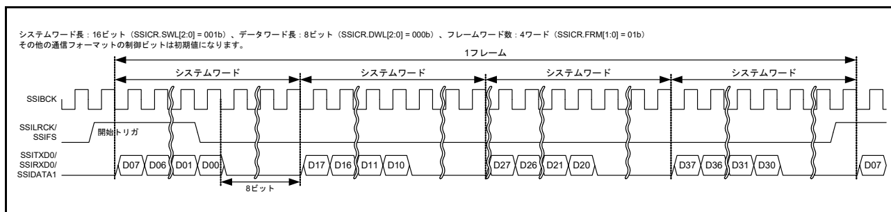
図 41.42 TDM フォーマット (パディングあり、システムワード長>データワード長)
