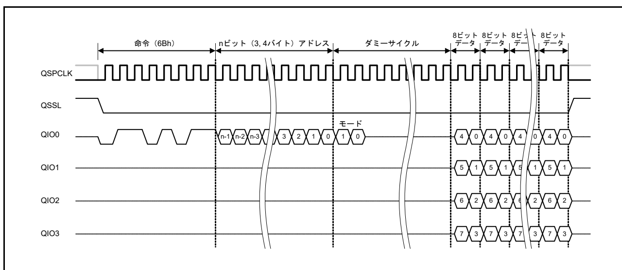
図 39.22 ファストリード Quad 出力バスサイクル
