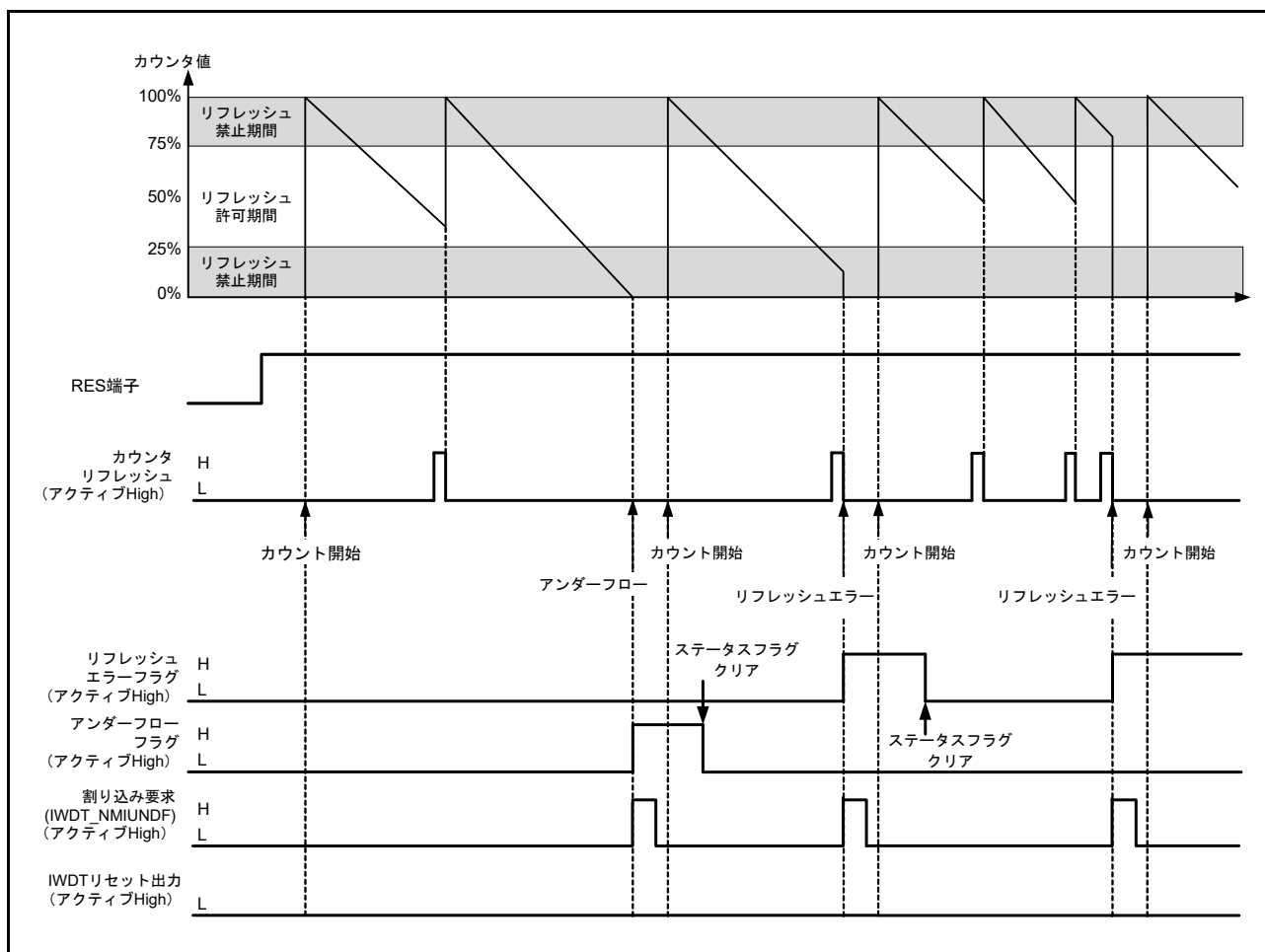
図 28.3 オートスタートモードでの動作例
