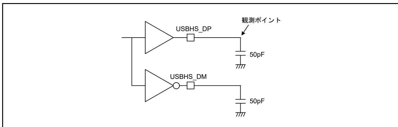
図 60.86 フルスピードモードにおける測定回路
