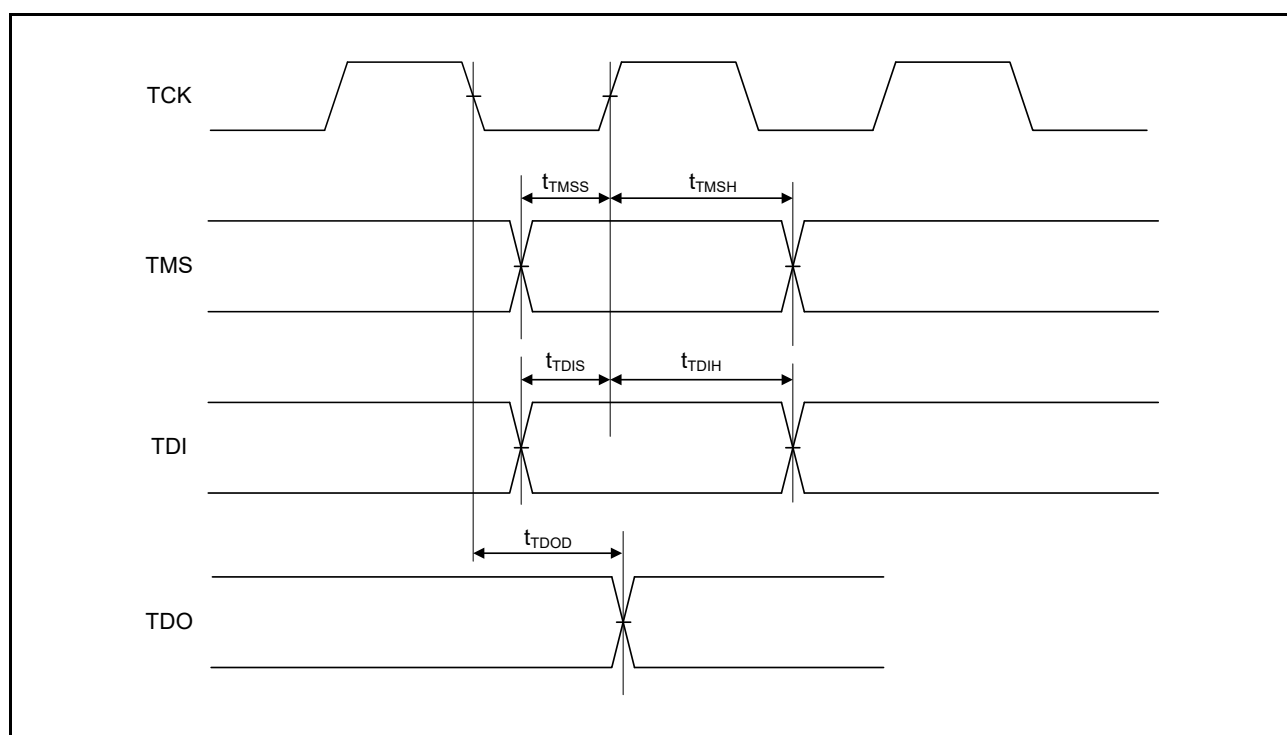
図 60.107 JTAG 入出力タイミング
