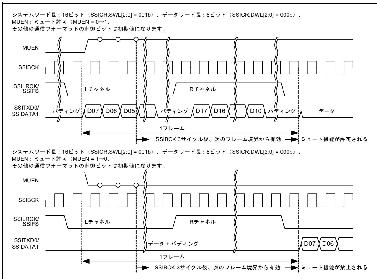
図 41.5 ミュート機能設定時の送信データ
