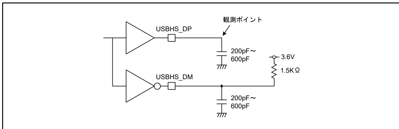
図 60.84 ロースピードモードにおける測定回路
