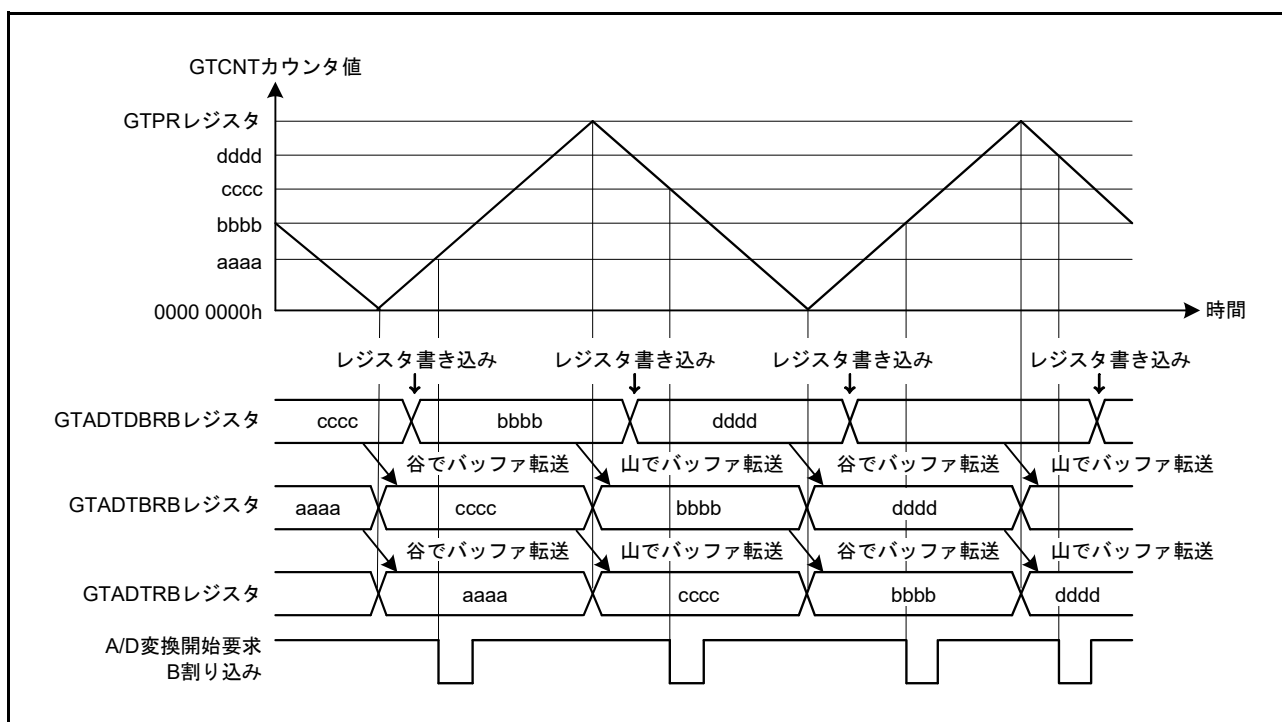
図 23.31 GTADTBRA、GTADTRB レジスタのダブルバッファ動作例 (三角波、谷と山の両方でバッファ転送、アップカウントとダウンカウント両方で A/D 変換開始要求割り込み発生の場合)
