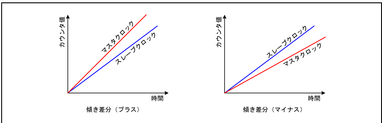
図 30.23 傾き差分の概念
