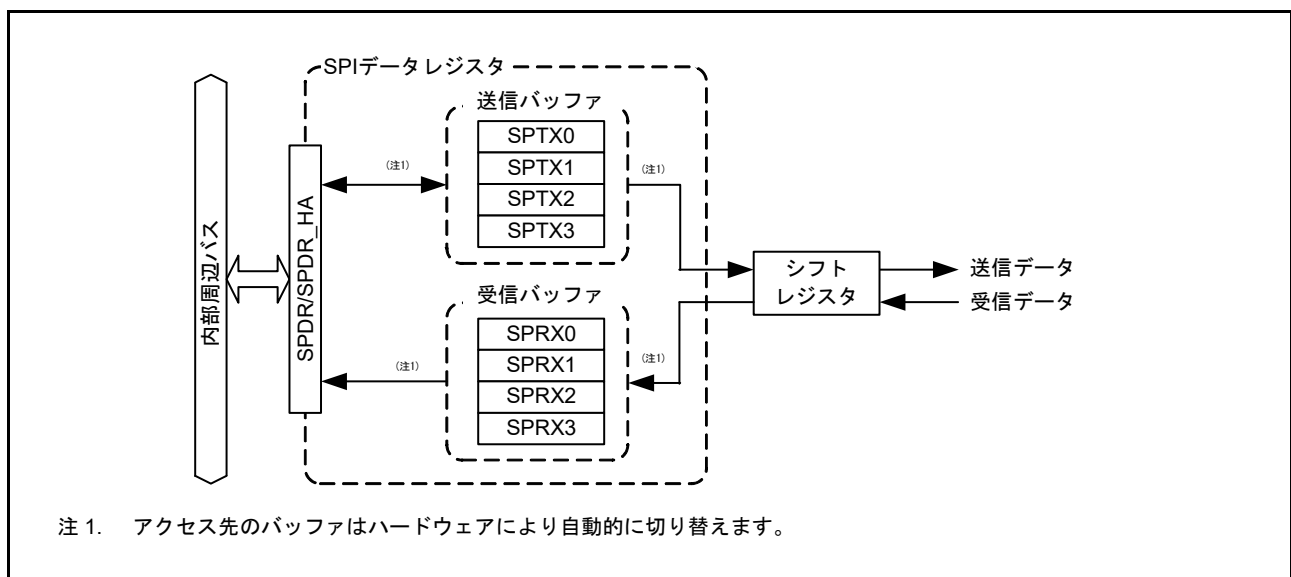
図 38.2 SPDR/SPDR_HA レジスタの構成図
