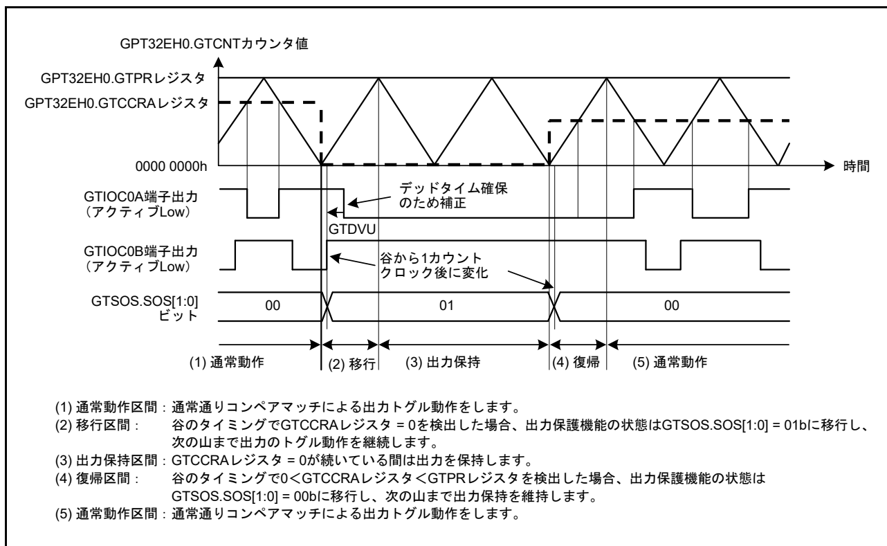
図 23.98 谷でのバッファ転送中に GTCCRA レジスタが 0 になった場合の出力保護機能の動作例 (谷でのバッファ転送中に 0 < GTCCRA レジスタ < GTPR レジスタを回復、アクティブ Low の場合)
