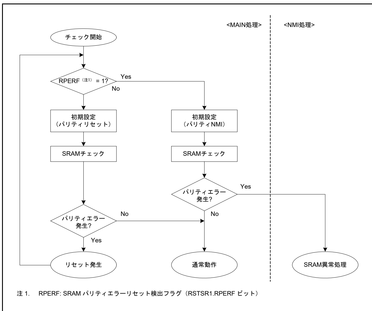
図 53.2 SRAM パリティリセット許可の場合の SRAM パリティチェックのフロー
