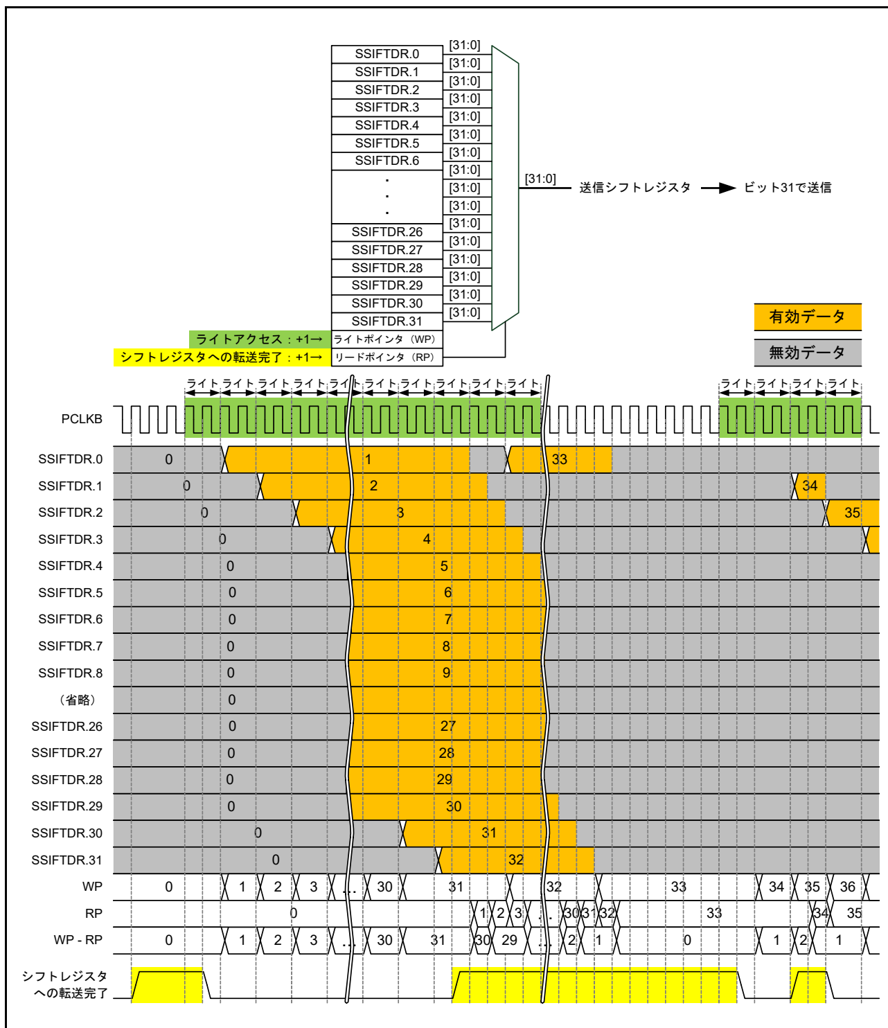
図 41.31 送信 FIFO データレジスタと送信シフトレジスタの構成および FIFO 動作例
