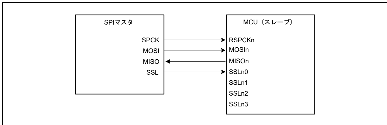
図 38.6 シングルマスタおよびシングルスレーブの構成例 (MCU はスレーブ、CPHA = 0)
