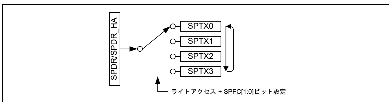
図 38.3 書き込み時の SPDR/SPDR_HA レジスタの構成図
