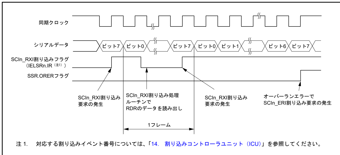
図 34.39 クロック同期式モードにおけるシリアル受信の動作例 (1) (RTS 機能を使用しない場合)
