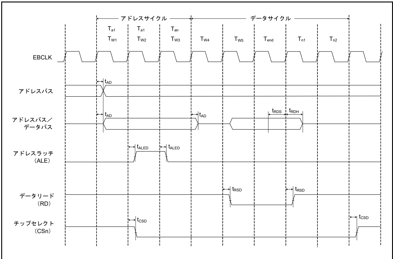
図 60.20 アドレス/データマルチプレクスバスのリードアクセスタイミング
