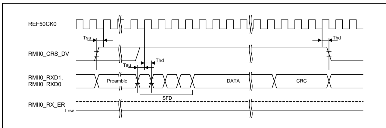
図 60.69 正常動作時の RMII 受信タイミング
