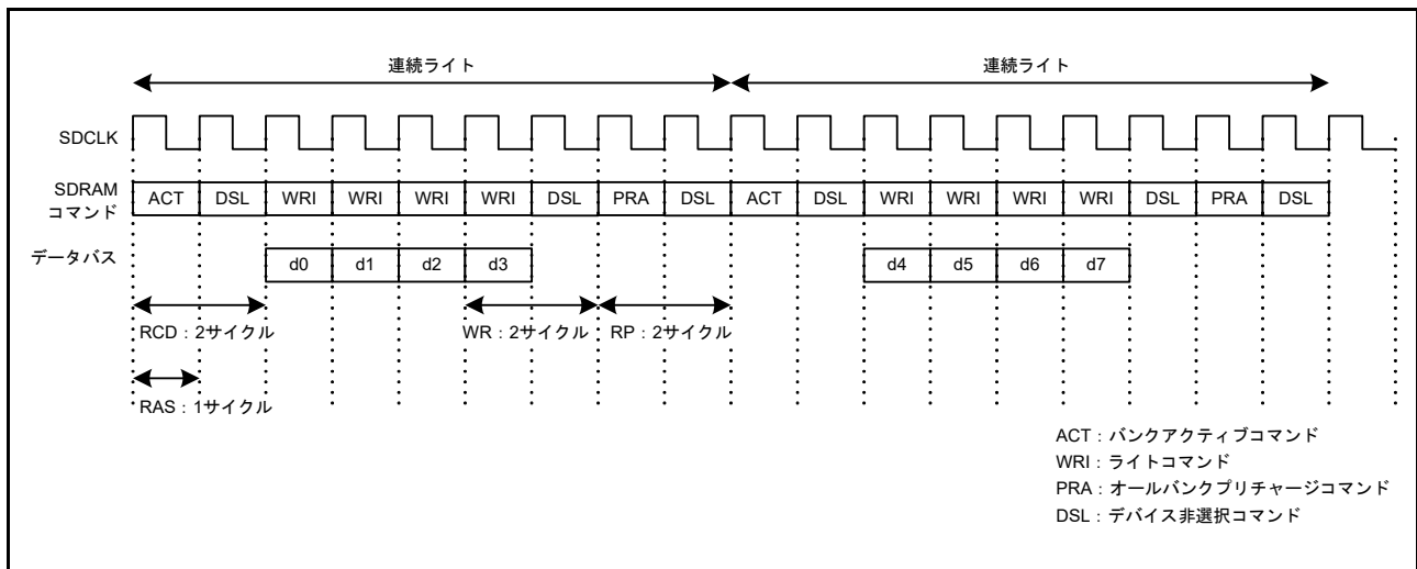
図 15.69 連続ライトタイミング例 (3)
