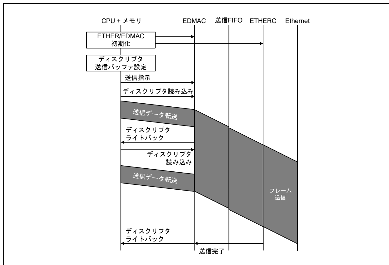
図 31.5 送信フローの例
