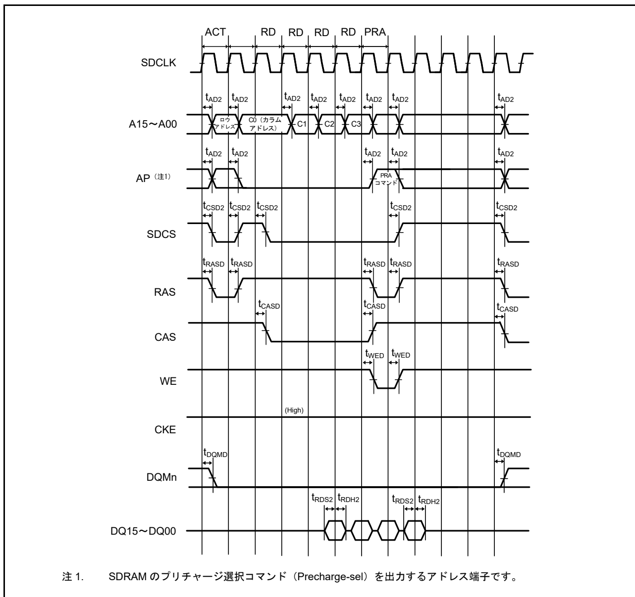
図 60.29 SDRAM 複数リードタイミング
