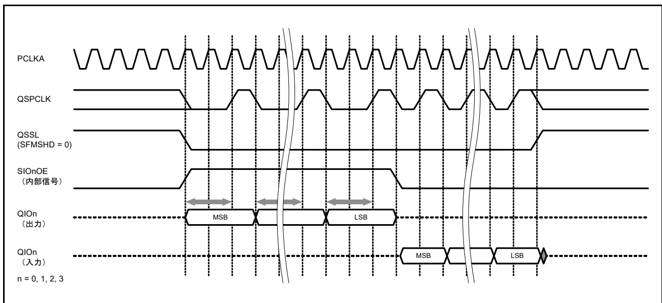
図 39.13 SFMOSW ビットを使用したシリアルデータ出力のセットアップ時間調整
