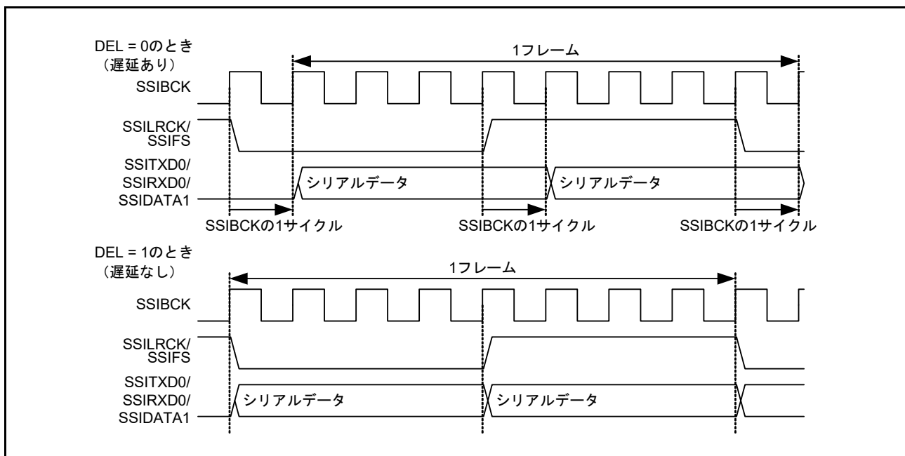
図 41.7 シリアルデータディレイの設定
