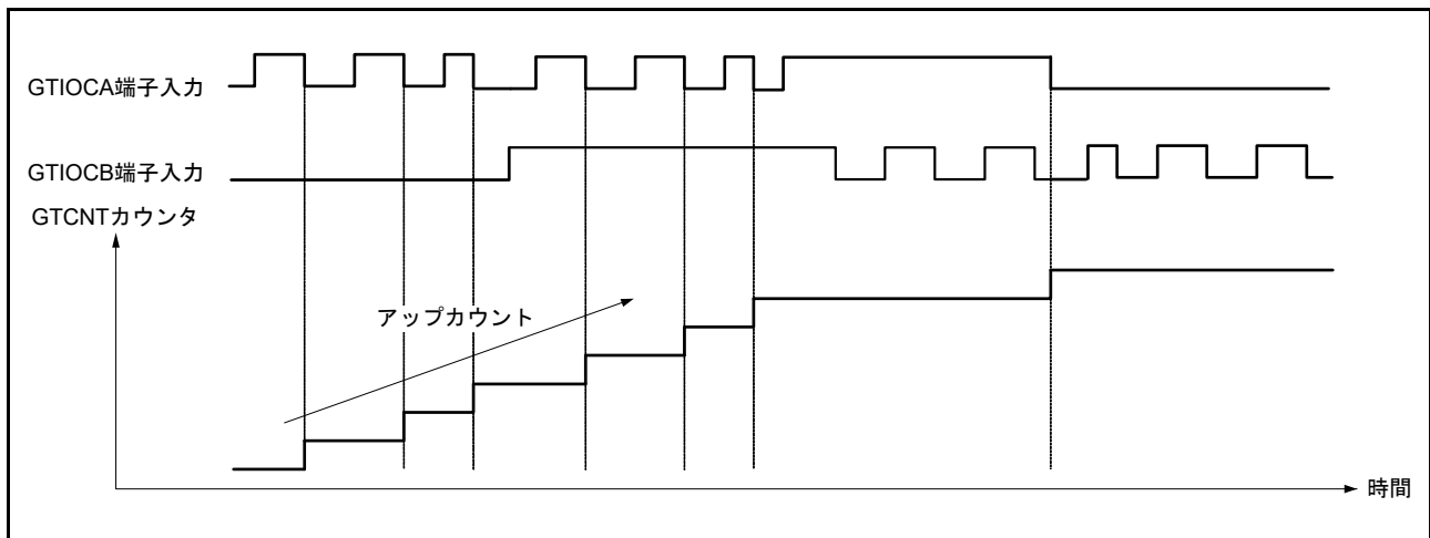
図 23.79 位相計数モード5の動作例 (A)
