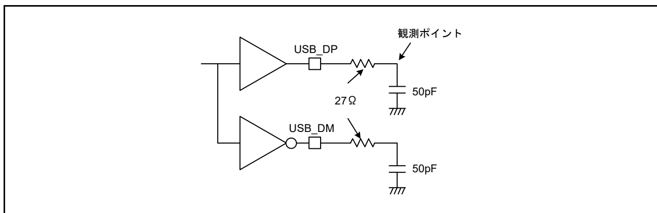
図 60.94 フルスピードモードにおける測定回路
