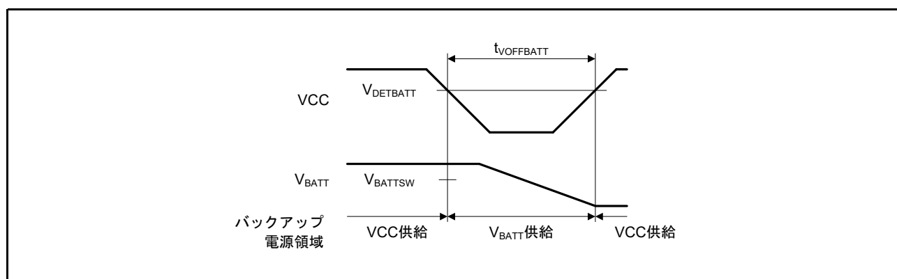
図 60.101 バッテリバックアップ機能特性
