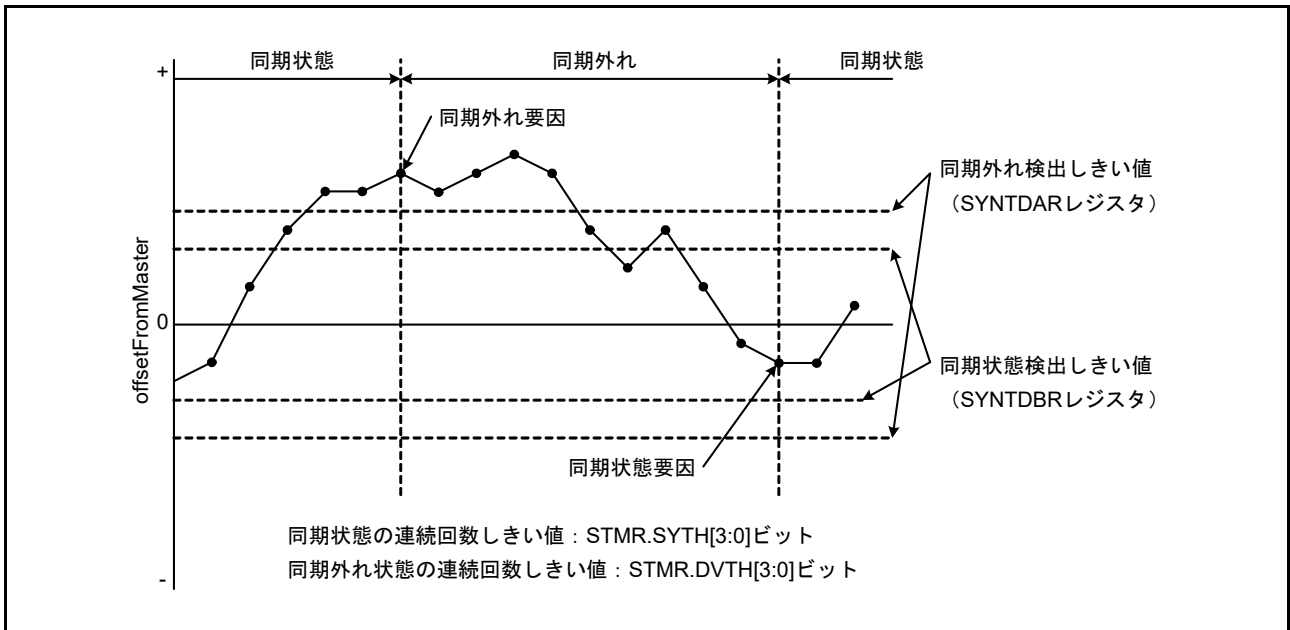
図 30.22 同期外れおよび同期状態の発生例 (STMR.DVTH[3:0] ビットおよび SYTH[3:0] ビットで連続検出回数を 3 回に指定)
