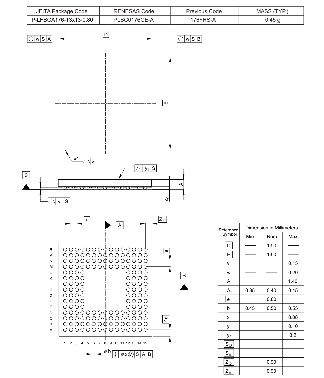
図 2.1 176-pin BGA
