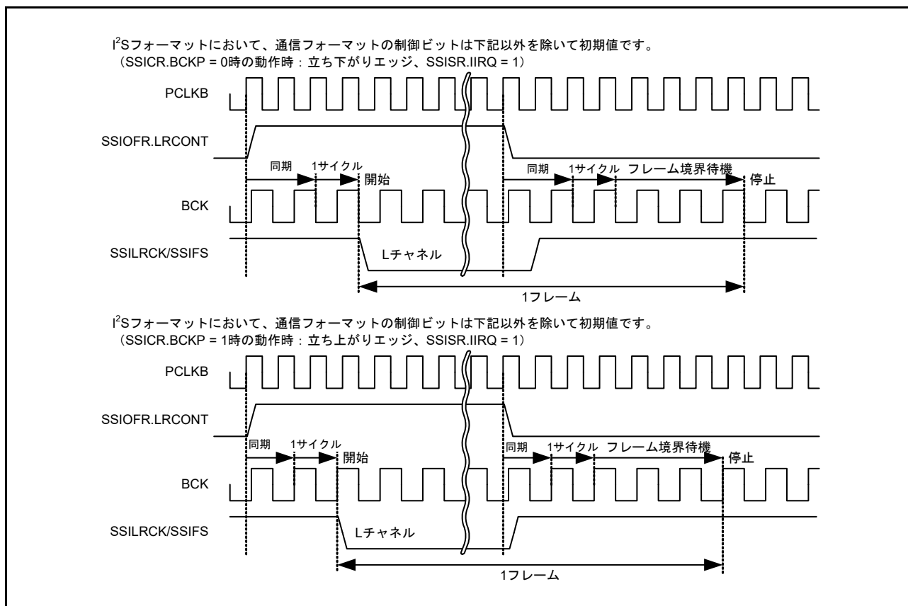
図 41.44 SSIOFR.LRCONT ビットによる LR クロック/フレーム同期継続の禁止例
