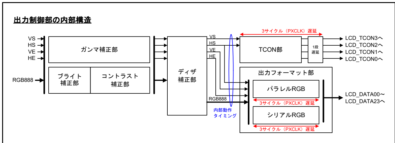
図 58.17 出力制御ブロックの内部構成
