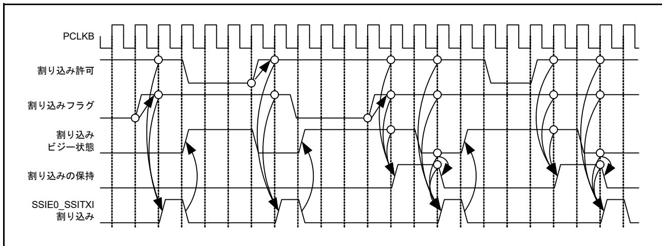
図 41.60 SSIE0_SSITXI 割り込みのタイミング図
