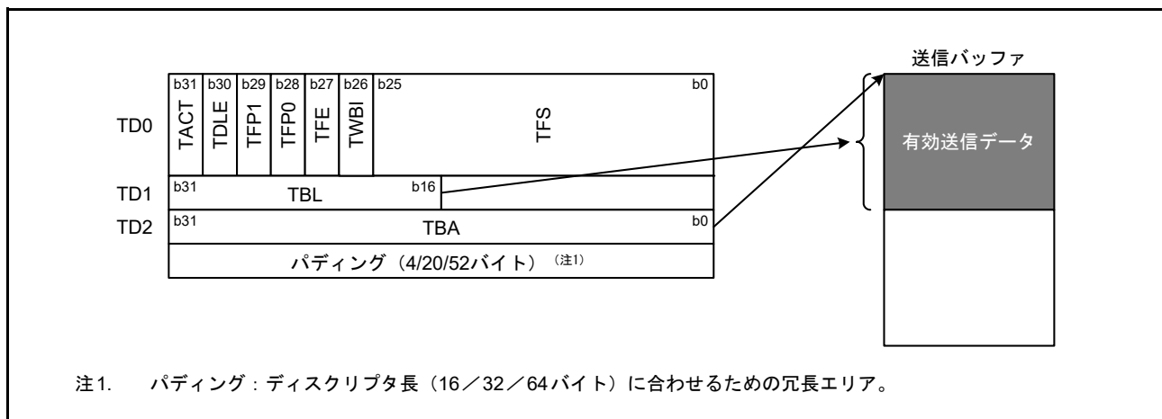
図 31.3 送信ディスクリプタと送信バッファの関係
