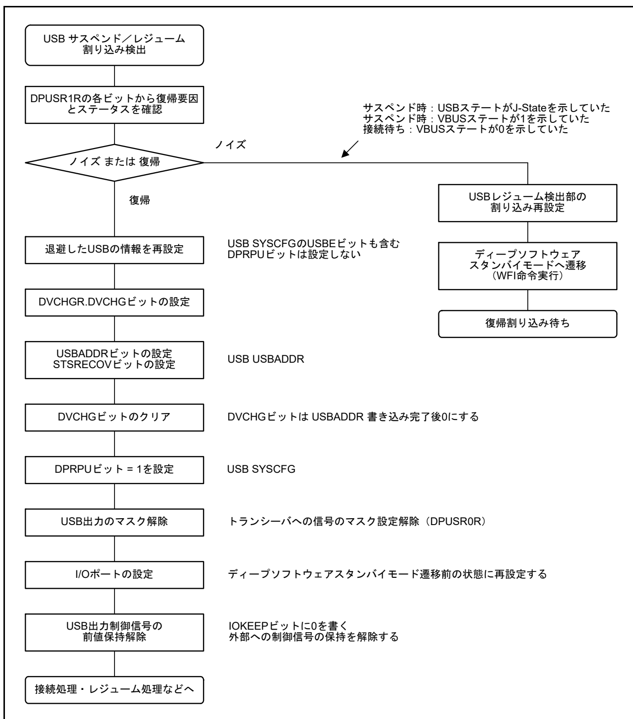
図 32.9 デバイスコントローラ機能選択時におけるディープソフトウェアスタンバイモード解除時の USBFS 設定フロー
