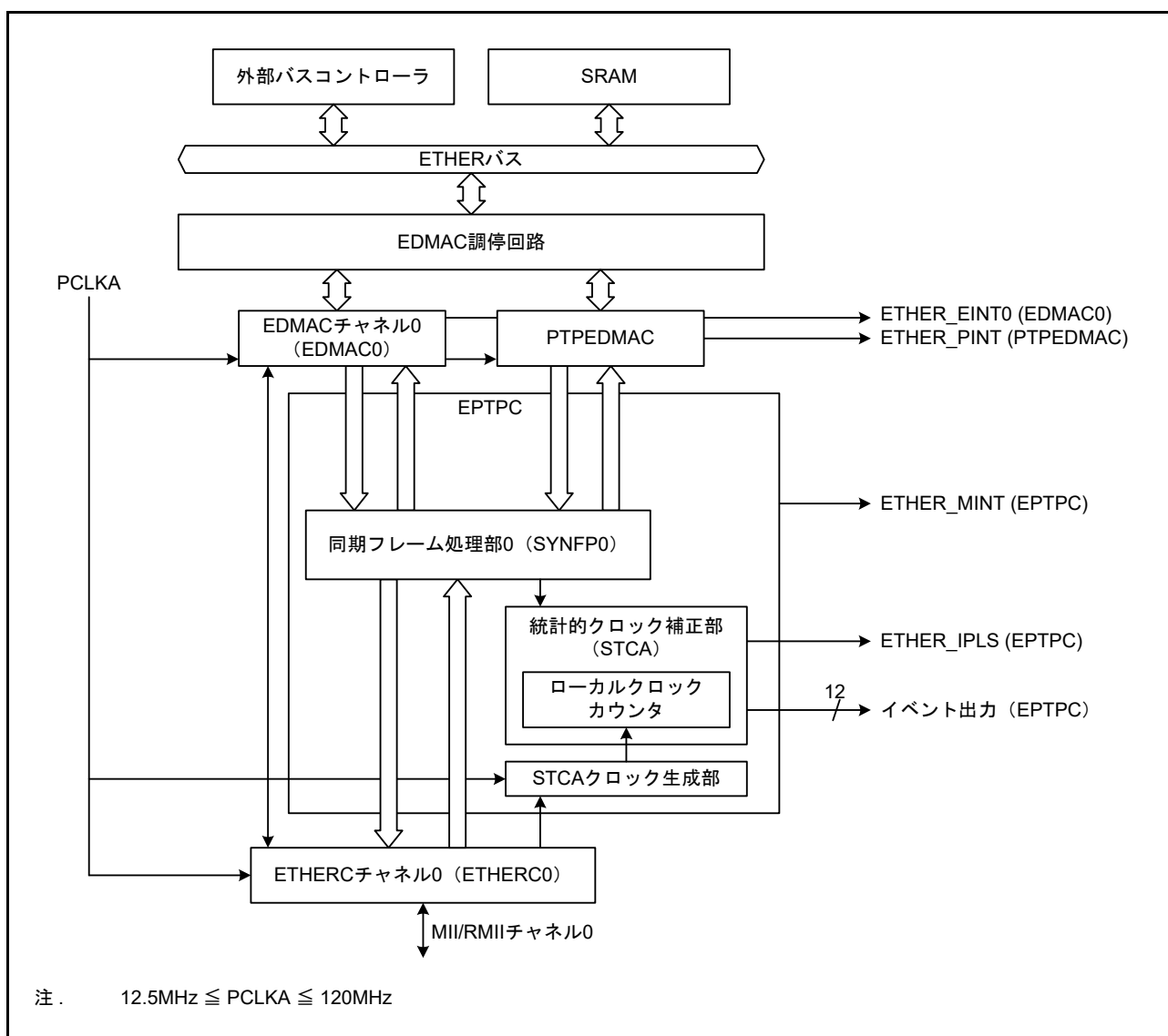
図 30.1 EPTPC の構成
