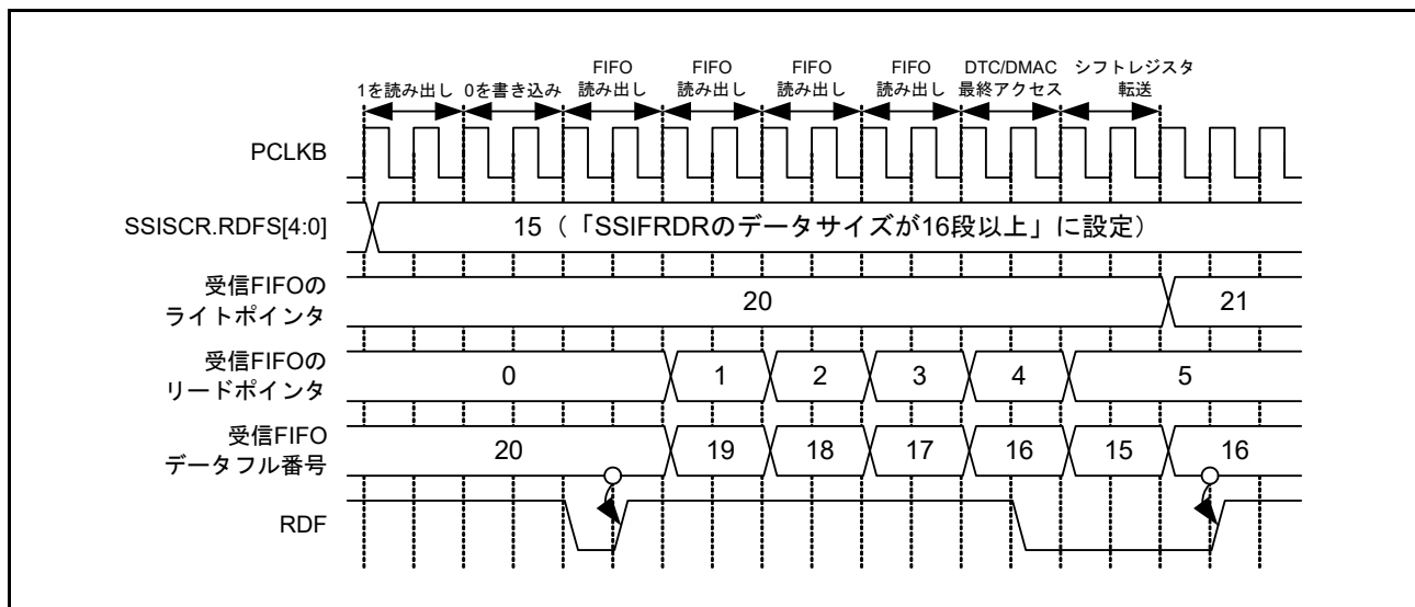
図 41.28 RDF の設定およびクリアのタイミング図
