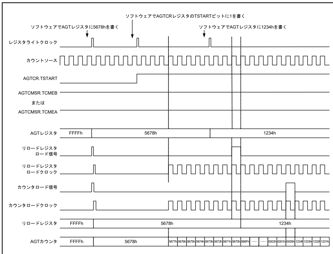
図 25.3 TSTART ビット値および TCMEA または TCMEB ビット値による書き換え動作のタイミング (コンペアマッチレジスタ A または B が有効の場合)
