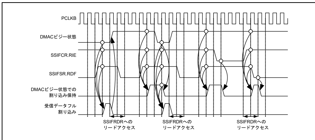
図 41.22 受信データフル割り込みのタイミング
