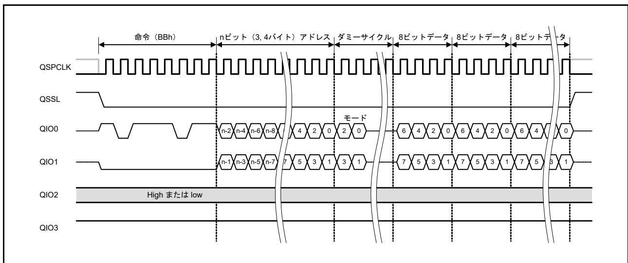
図 39.20 ファストリード Dual I/O バスサイクル
