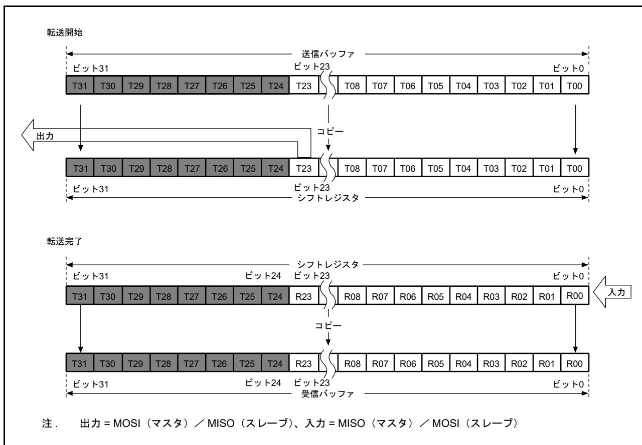
図 38.15 MSB ファースト転送 (24 ビットデータ/パリティ機能無効)
