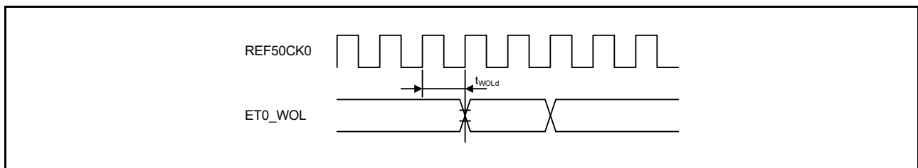
図 60.71 RMI0 に対する WOL 出力タイミング
