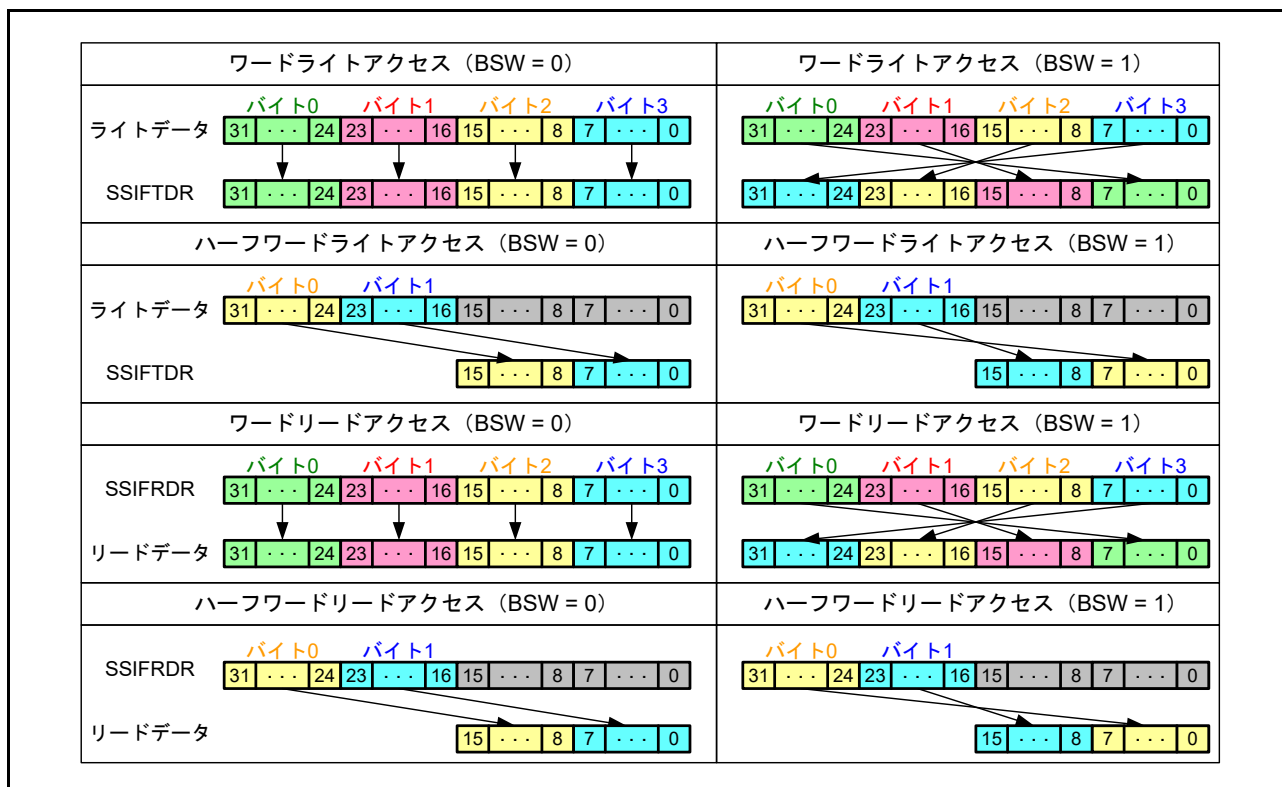
図 41.24 バイトスワップの動作例
