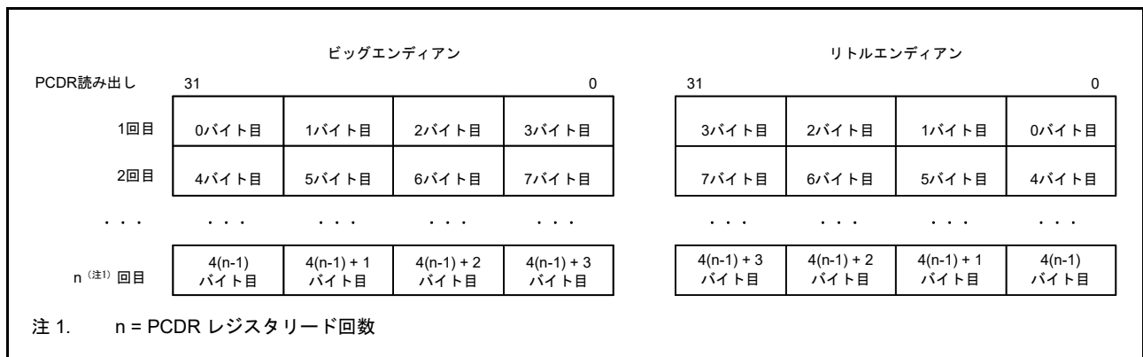
図 44.3 エンディアンフォーマット
