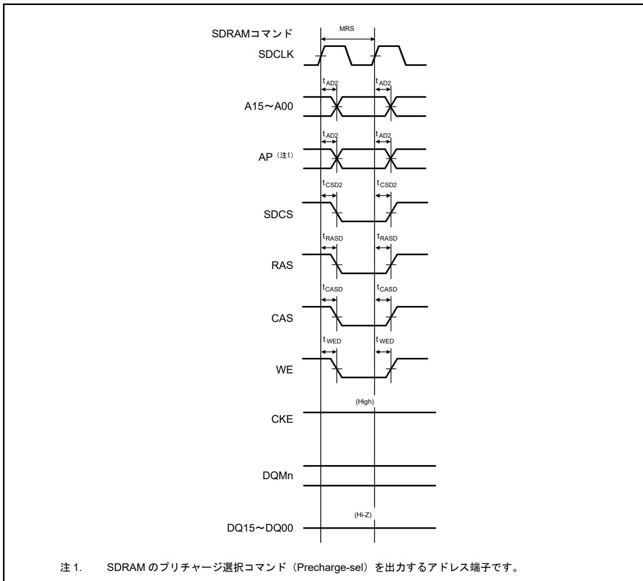
図 60.32 SDRAM モードレジスタセットタイミング
