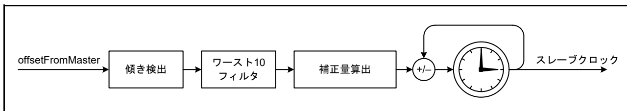
図 30.20 時刻補正回路の構成
