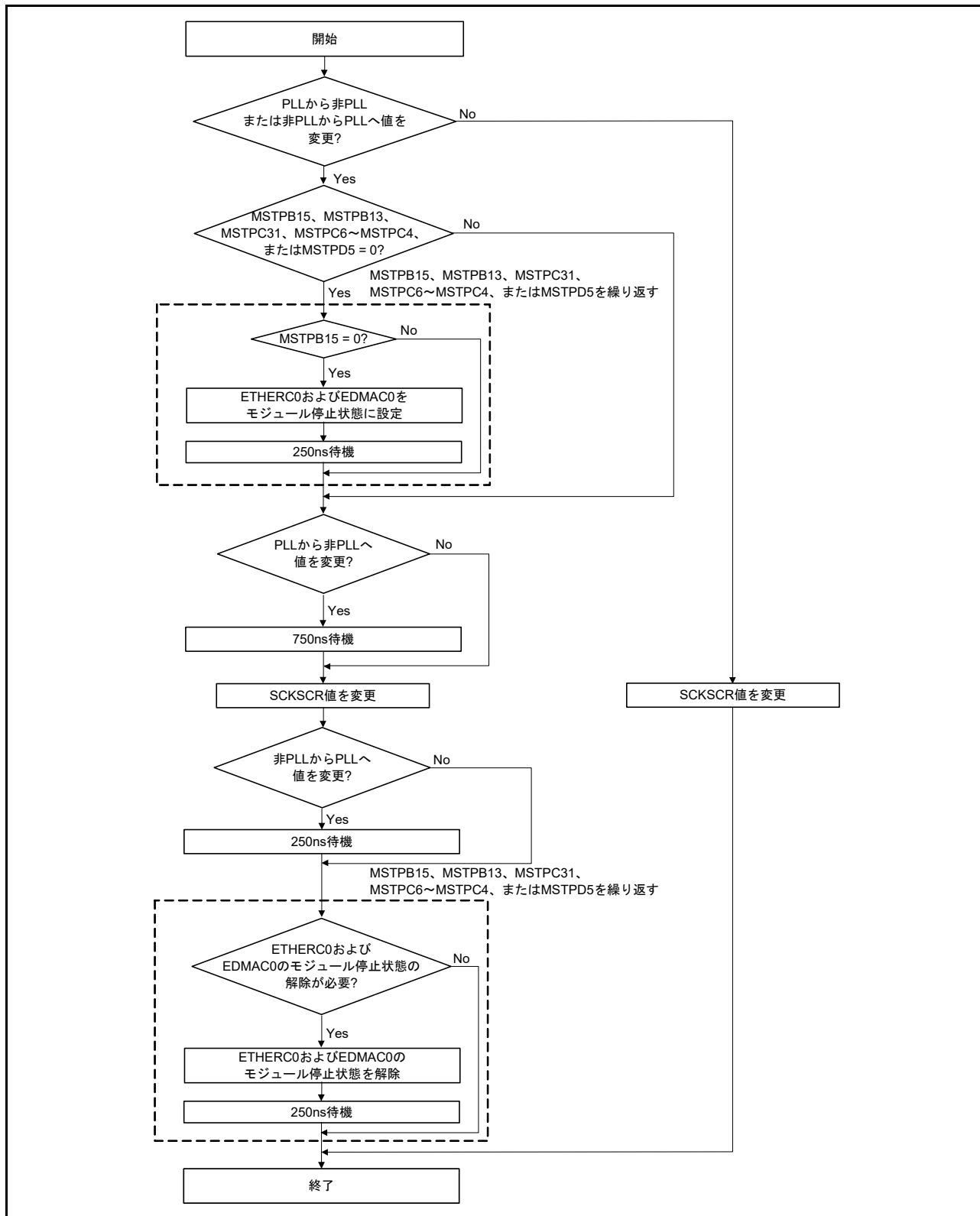
図 9.3 SCKSCR 値変更のフロー例
