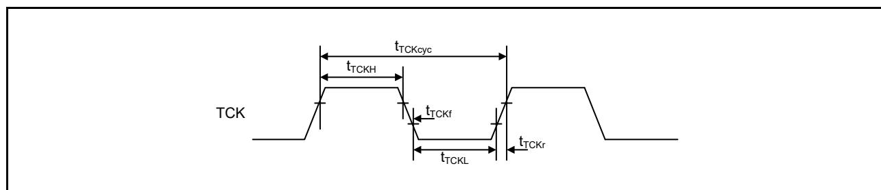
図 60.103 バウンダリスキャン TCK タイミング
