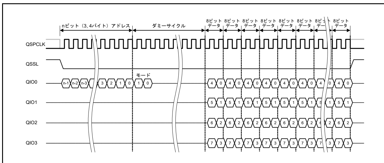
図 39.23 XIP モード時のファストリード Quad 出力バスサイクル
