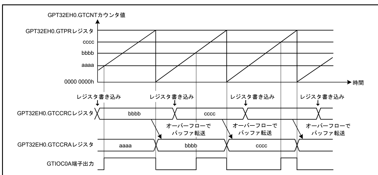
図 23.22 GTCCRA、GTCCRB レジスタのバッファ動作例 (アウトプットコンペア、アップカウント時ののこぎり波、GTCCRA レジスタのコンペアマッチで High 出力、周期の終わりで Low 出力の場合)
