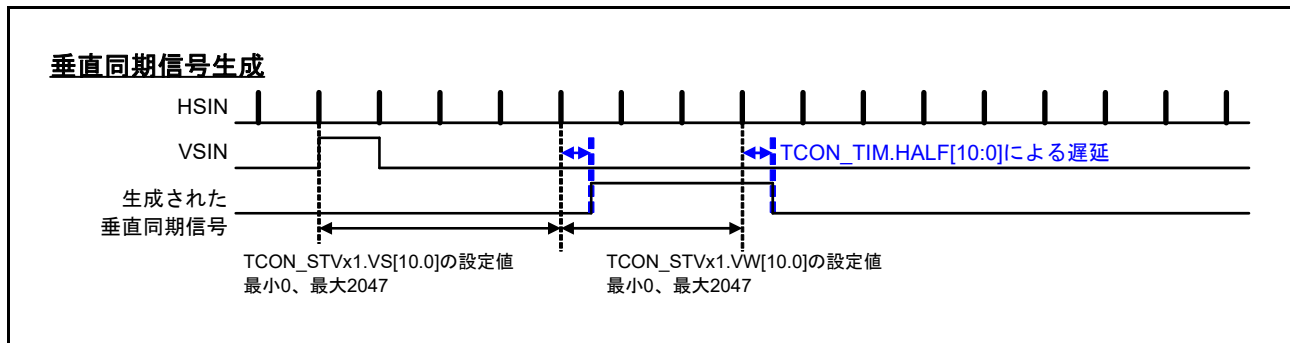
図 58.18 垂直同期信号の生成
