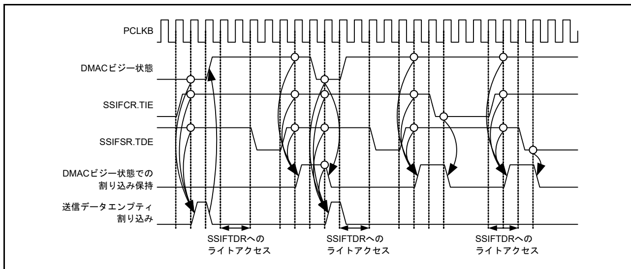
図 41.23 送信データエンプティ割り込みのタイミング
