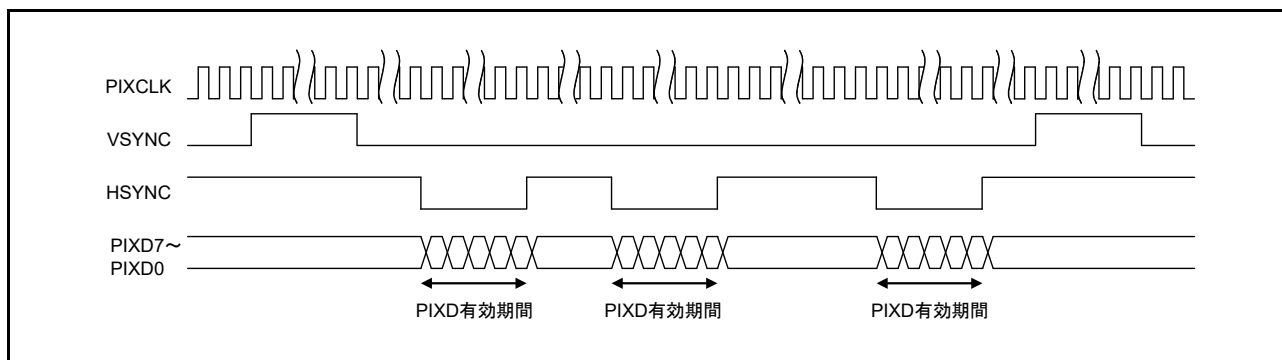
図 44.7 VPS = 1、HPS = 1 の場合の PDC 転送フォーマット
