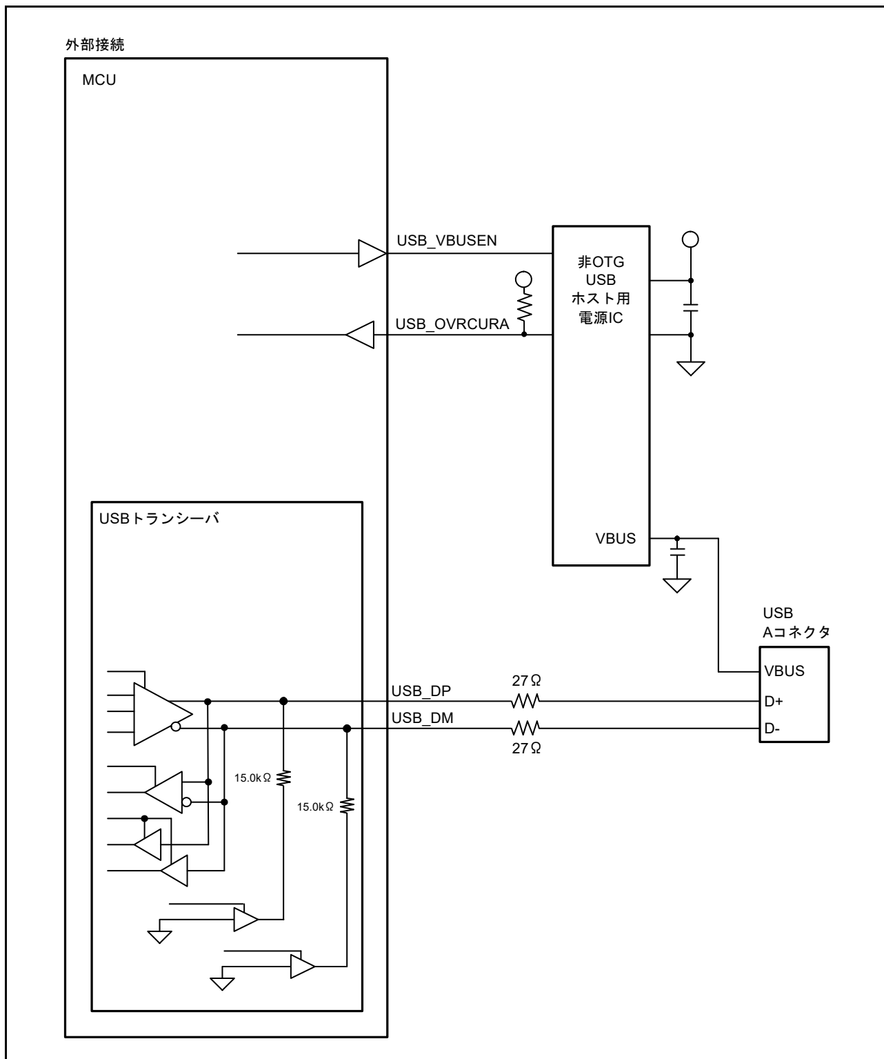
図 32.4 ホスト接続例
