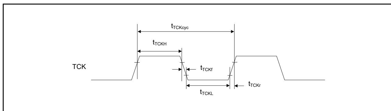
図 60.106 JTAG TCK タイミング
