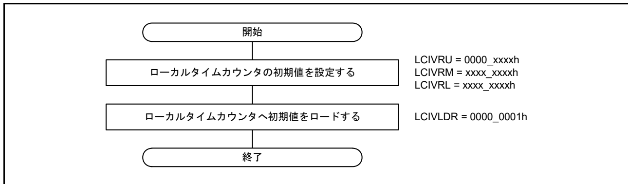
図 30.26 ローカルクロックカウンタへの初期値設定の手順
