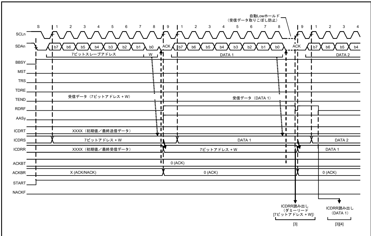
図 36.19 スレーブ受信の動作タイミング (1) (7 ビットアドレスフォーマットで RDRFS = 0 の場合)
