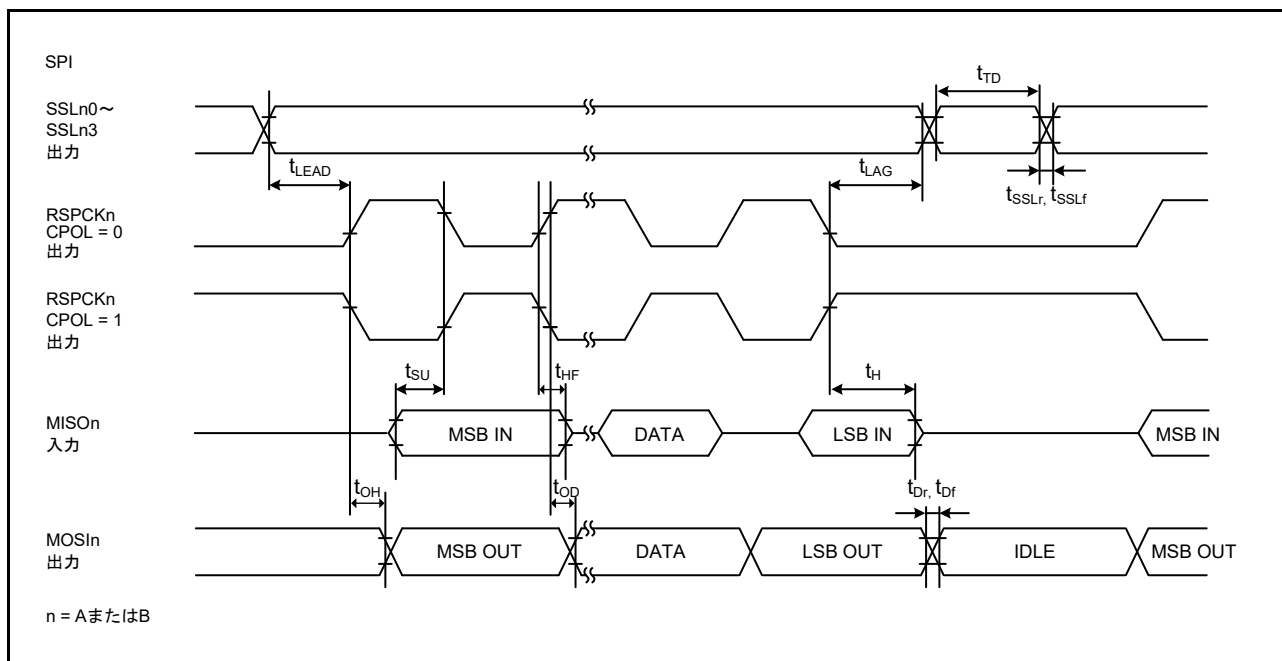
図 60.55 CPHA = 1 で、PCLKA/2 にビットレートが設定されている場合におけるマスタの SPI タイミング
