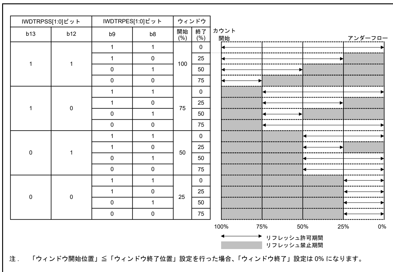
図 28.2 IWDTRPSS[1:0] および IWDTRPES[1:0] ビットとリフレッシュ許可期間
