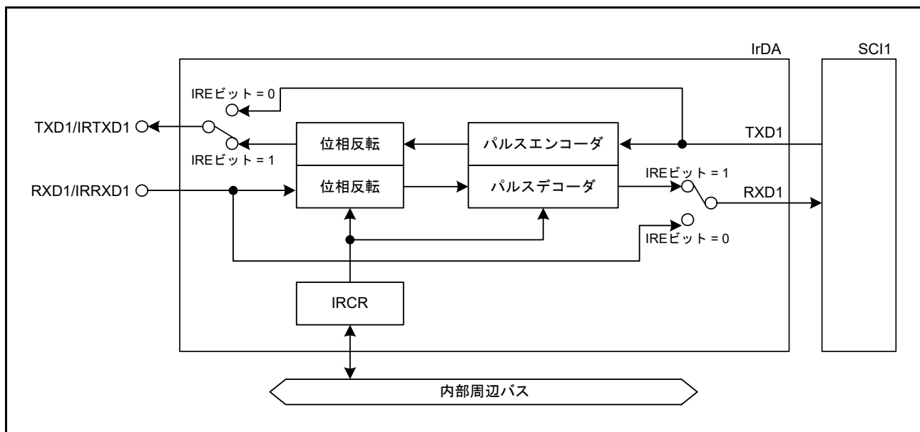
図 35.1 IrDA インタフェースと SCI1 の連携
