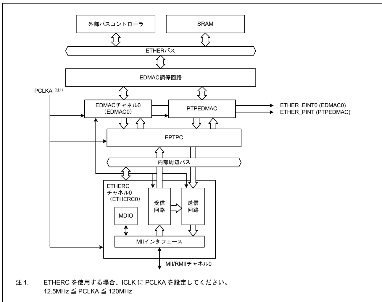
図 29.1 ETHERC の構成
