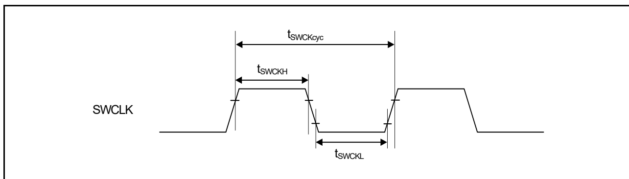
図 60.108 SWD SWCLK タイミング
