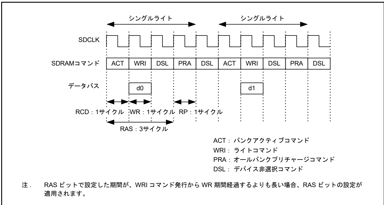
図 15.62 シングルライトタイミング例 (4)
