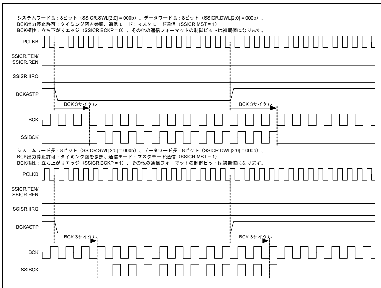
図 41.34 BCKASTP ビットの動作例 (アイドル状態の場合)
