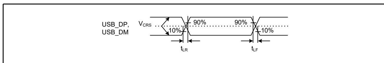
図 60.91 ロースピードモードにおけるUSB_DP、USB_DMの出力タイミング
