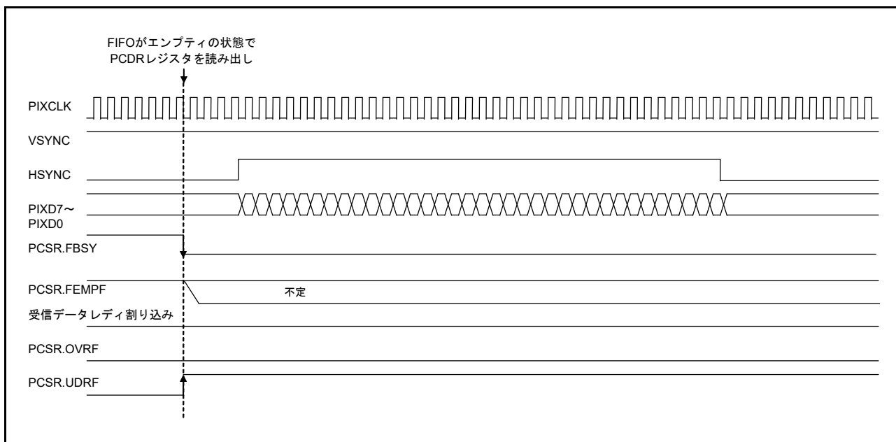
図 44.15 アンダーラン検出時の動作
