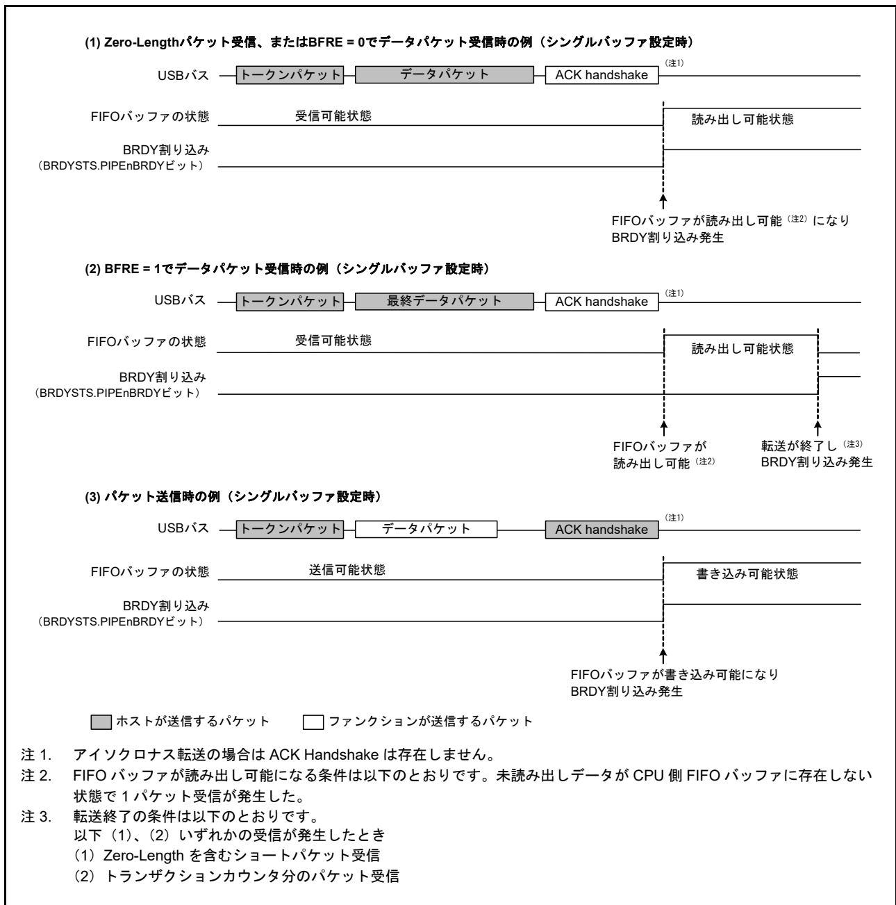
図 32.11 BRDY 割り込み発生タイミング
