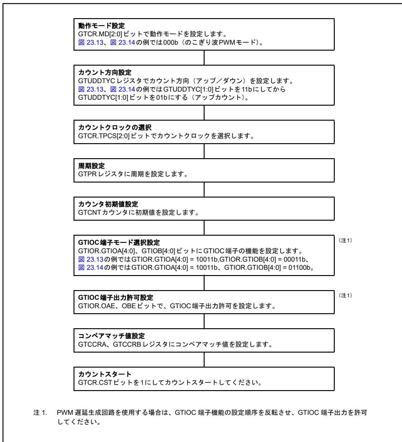
図 23.15 トル出力動作設定例
