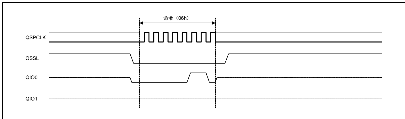
図 39.28 ライトイネーブルバスサイクル
