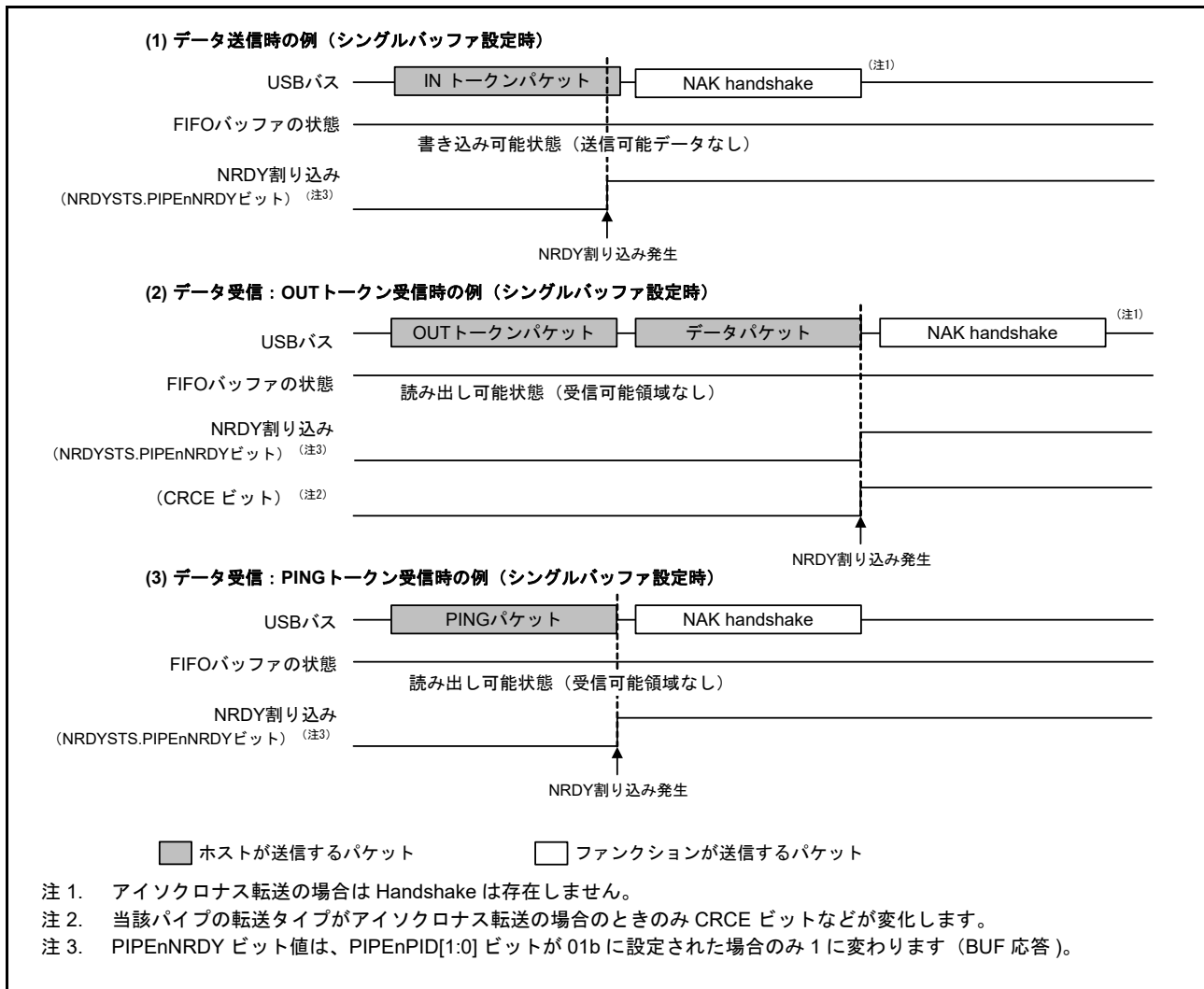
図 32.12 デバイスコントローラモード時の NRDY 割り込み発生タイミング
