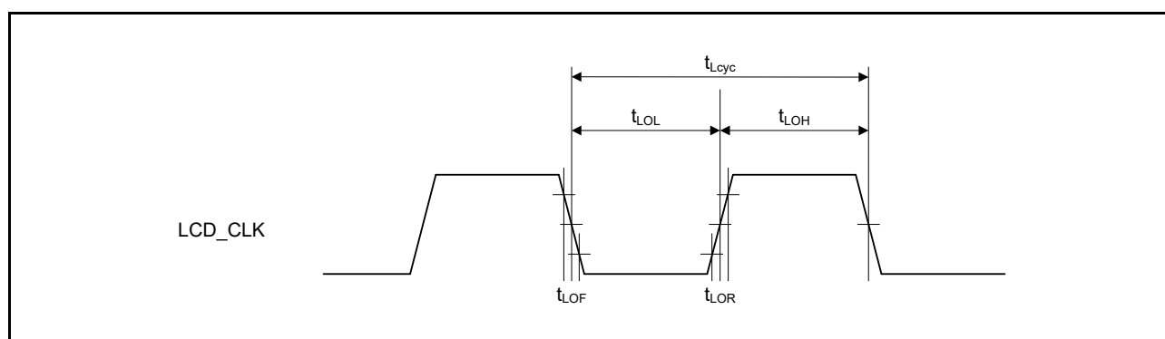
図 60.81 LCD_CLK クロック出カタイミング
