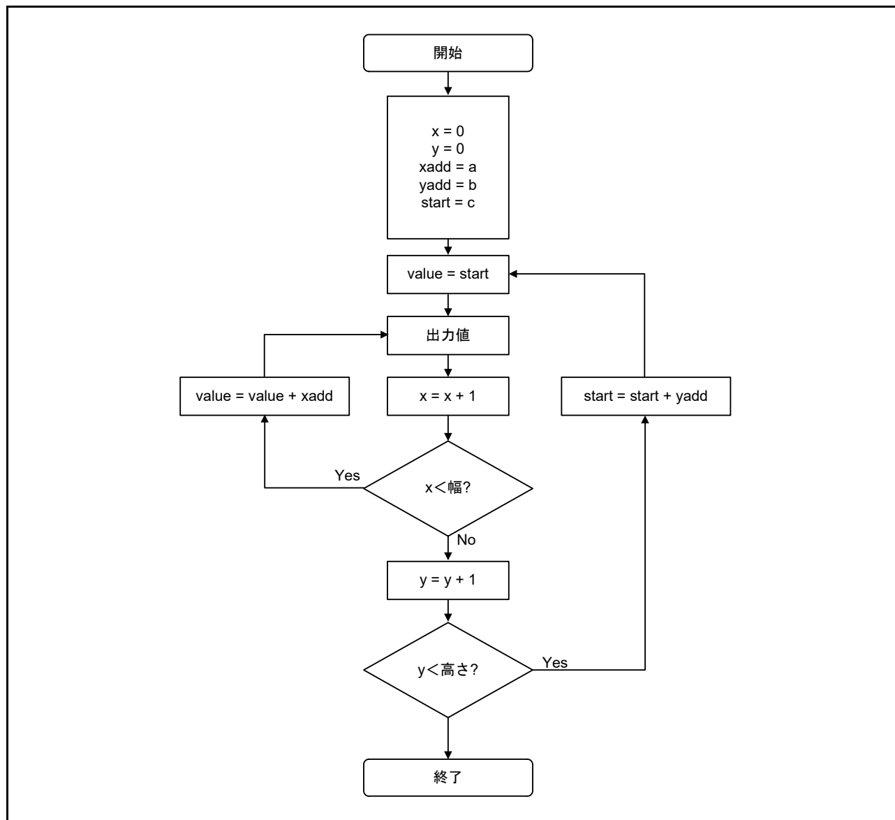
図 56.8 線形リミッタの動作フロー
