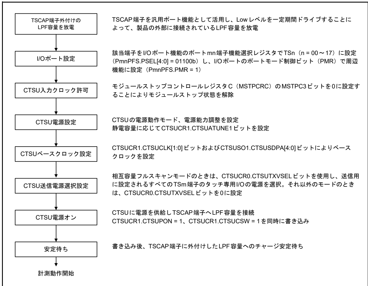
図 51.9 CTSUS 初期設定フロー
