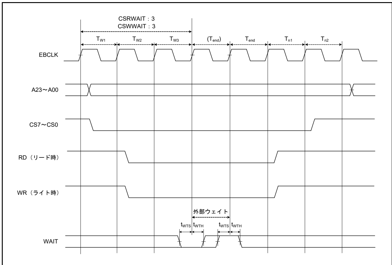
図 60.26 外部ウェイト制御の外部バスタイミング
