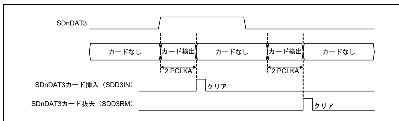
図 43.8 SDnDAT3 による SD カード検出
