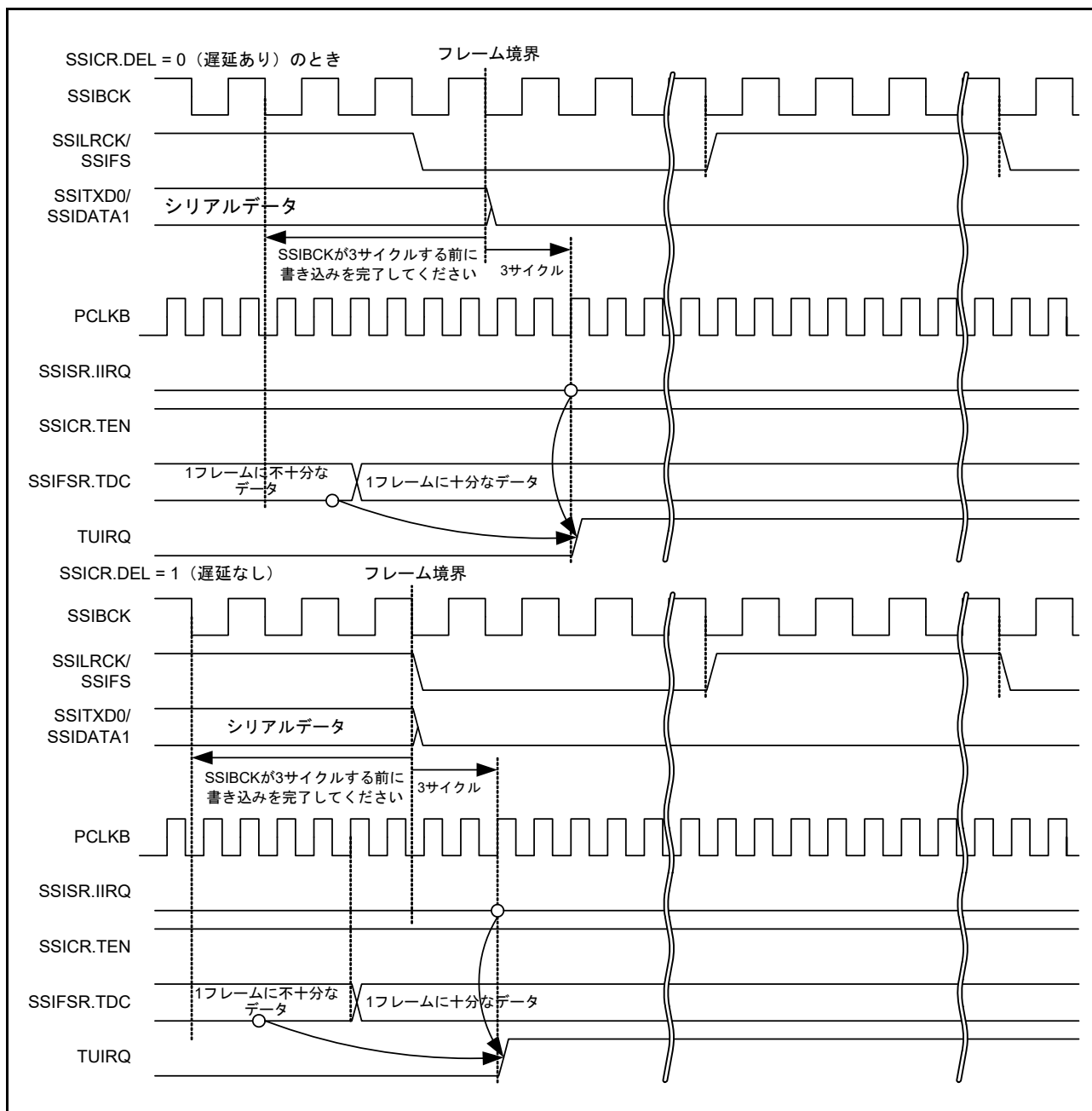
図 41.20 TUIRQ 設定タイミング (通信が継続する場合)
