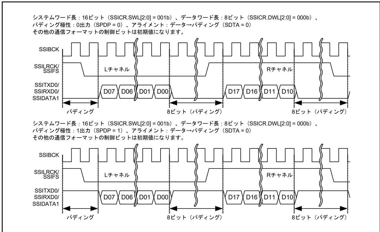
図 41.11 パディングビット極性
