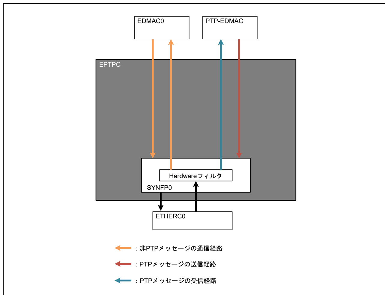
図 30.3 フレーム転送に関するモジュールのブロック図
