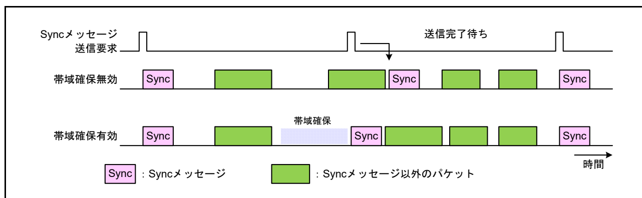
図 30.31 Syncメッセージ送信帯域の確保
