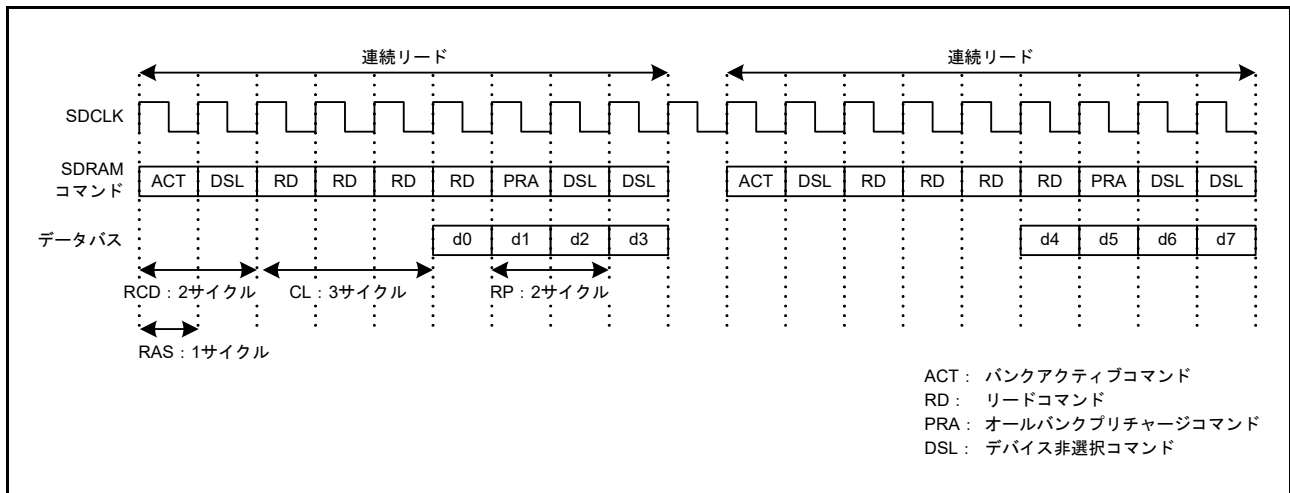
図 15.66 連続リードタイミング例 (3)
