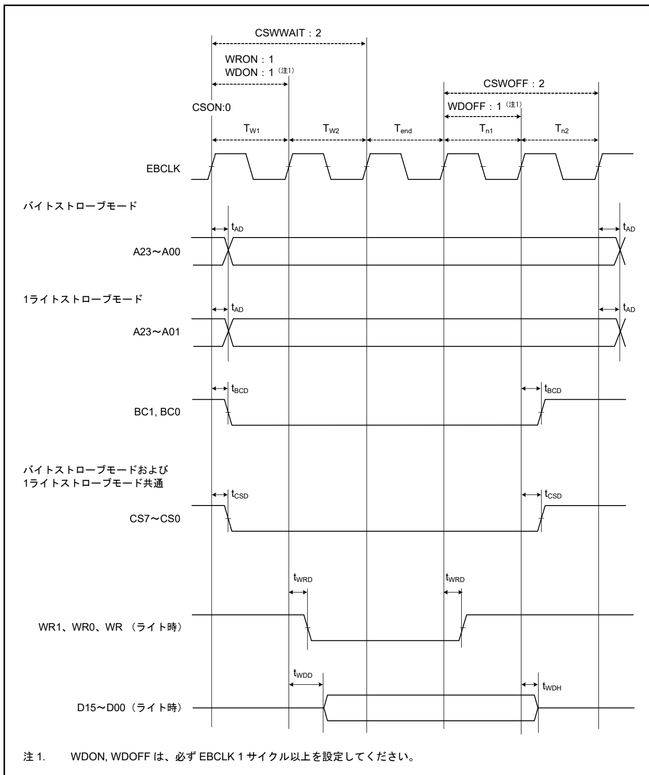
図 60.23 バスクロック同期を使用したノーマルライトサイクルの外部バスタイミング
