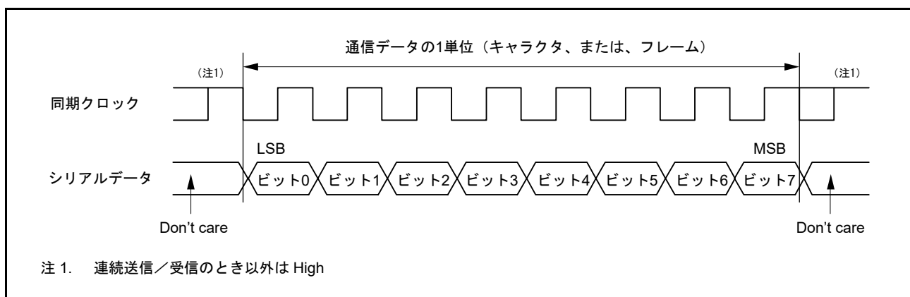
図 34.31 クロック同期式シリアル通信のデータフォーマット (LSB ファーストの並び順の場合)
