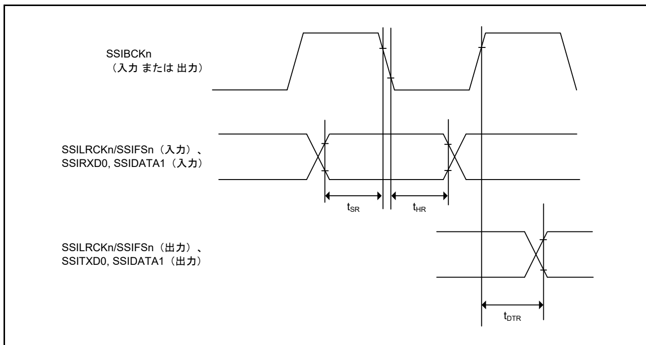
図 60.64 SSICR.BCKP = 1 の場合の SSIE データ送受信タイミング
