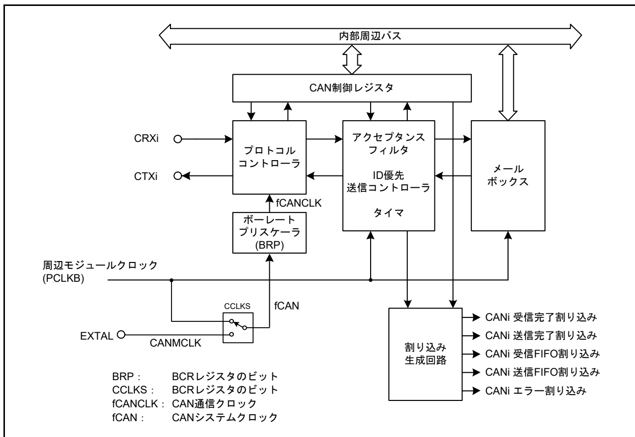
図 37.1 CANモジュールブロック図 (i = 0, 1)
