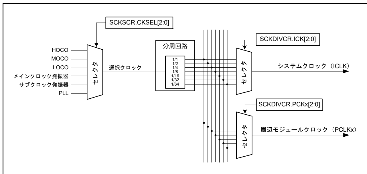
図 9.13 クロックソース選択ブロック図
