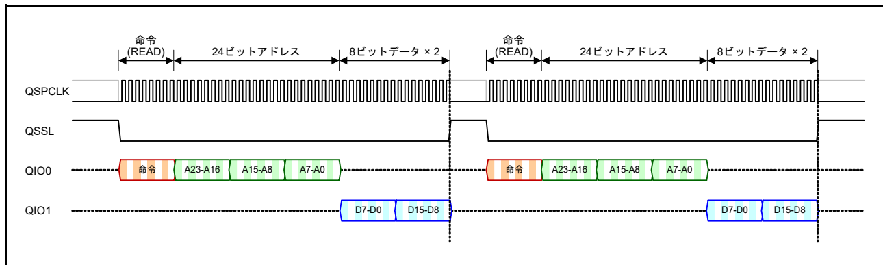
図 39.29 個々の変換に基づく連続データリード動作
