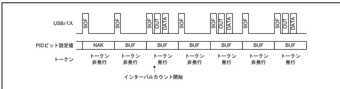
図 32.17 IITV = 1 の場合のトークン発行の有無
