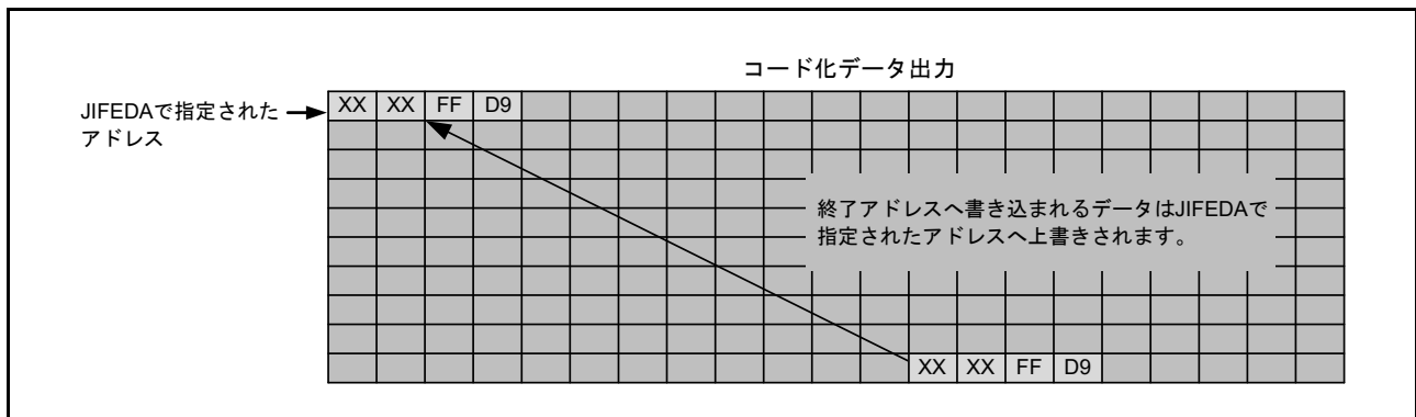
図 57.3 出力符号データ異常転送の概念図
