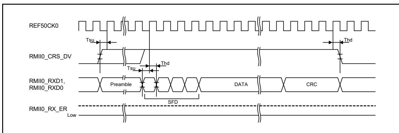
図 60.69 正常動作時の RMII 受信タイミング
