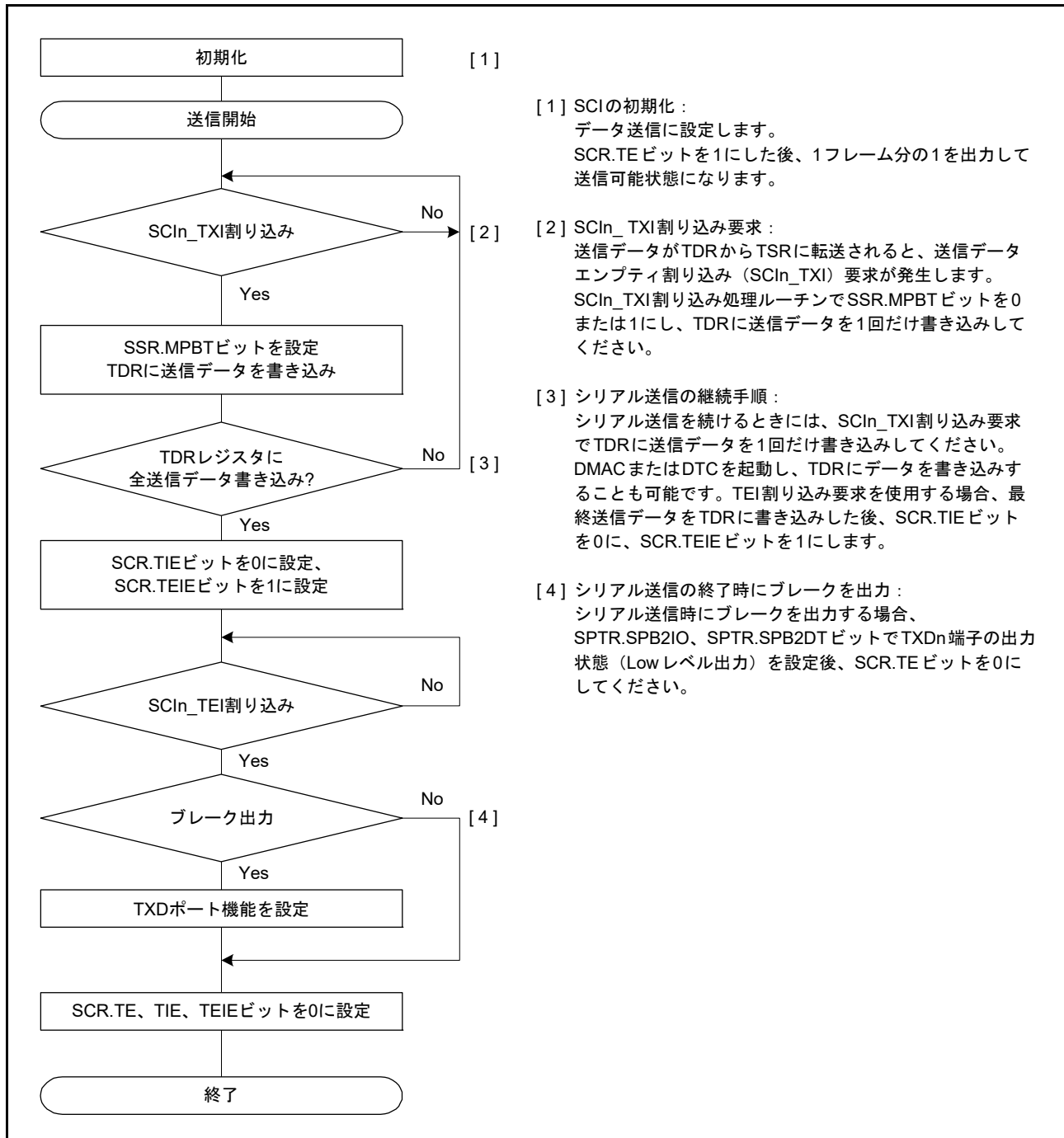
図 34.23 マルチプロセッサシリアル送信のフローチャート例 (非 FIFO 選択時)
