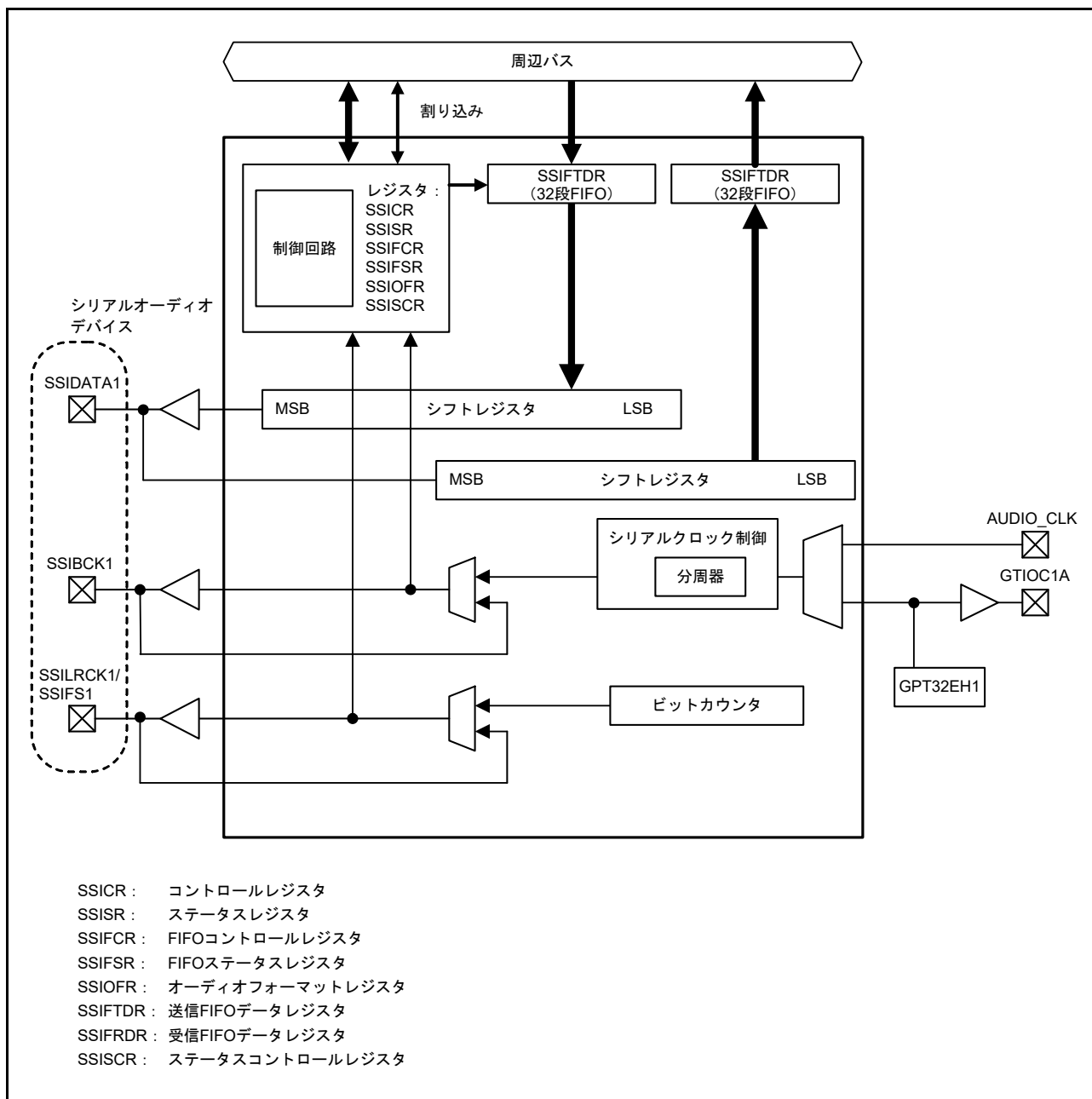
図 41.3 SSIE ブロック図 (SSIE1)
