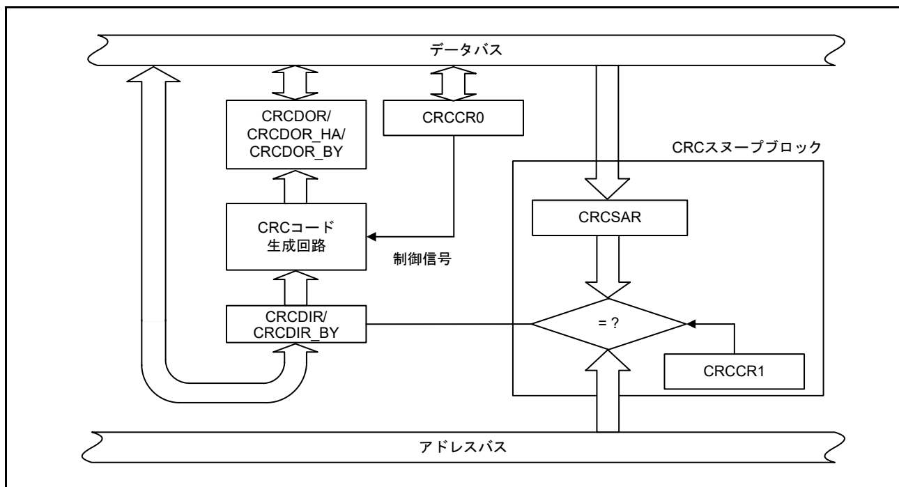
図 40.1 CRC 演算器のブロック図
