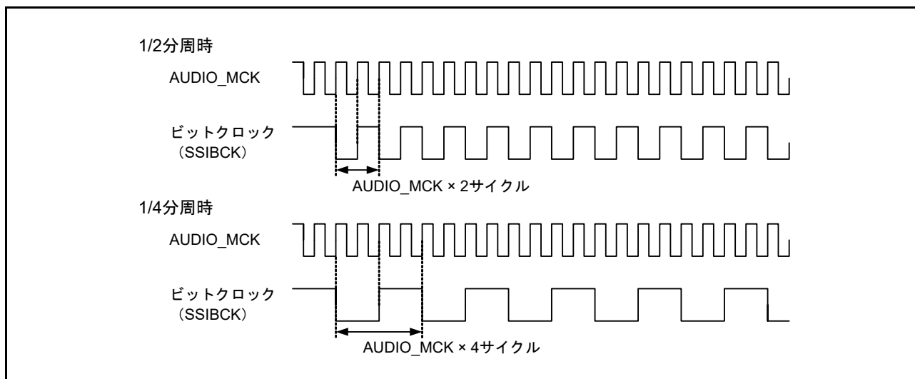
図 41.6 マスタモード通信時のサンプリング周波数
