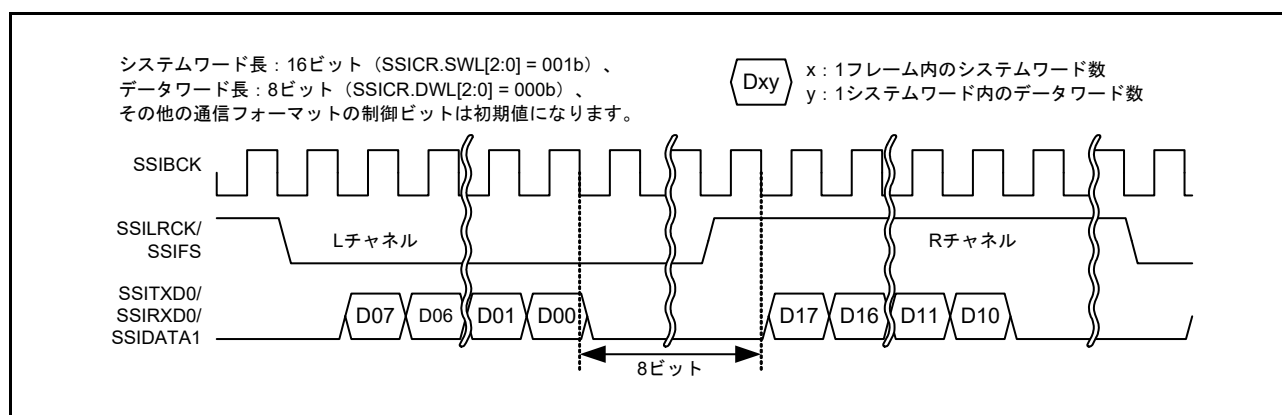
図 41.36 パディングビットの転送例 (I 2 S フォーマット、システムワード長>データワード長)
