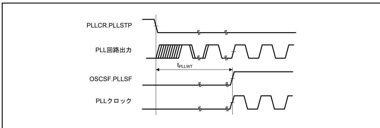
図 60.11 PLL クロック発振開始タイミング
