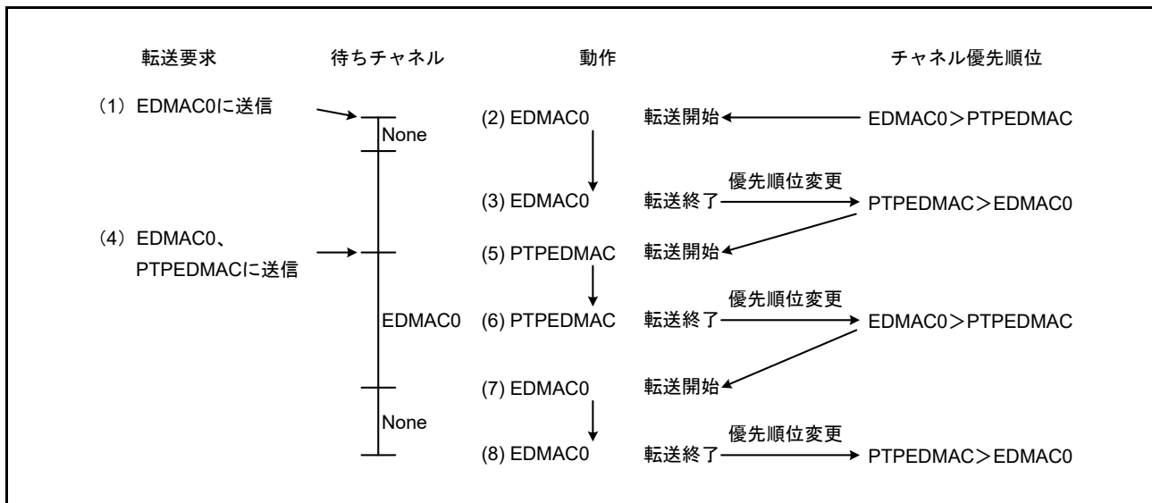
図 31.10 チャンネル優先順位変更の例
