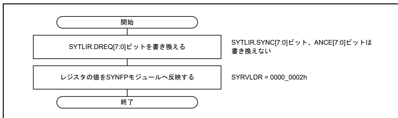
図 30.9 Delay_Resp メッセージの logMessageInterval フィールド値の変更手順
