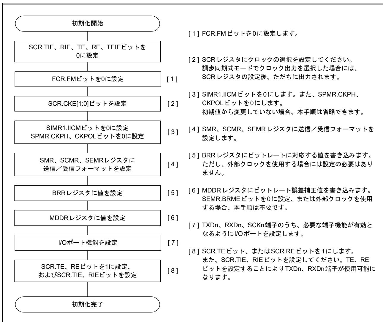
図 34.7 調歩同期式モードにおける SCI の初期化フローチャート例（非 FIFO 選択時）
