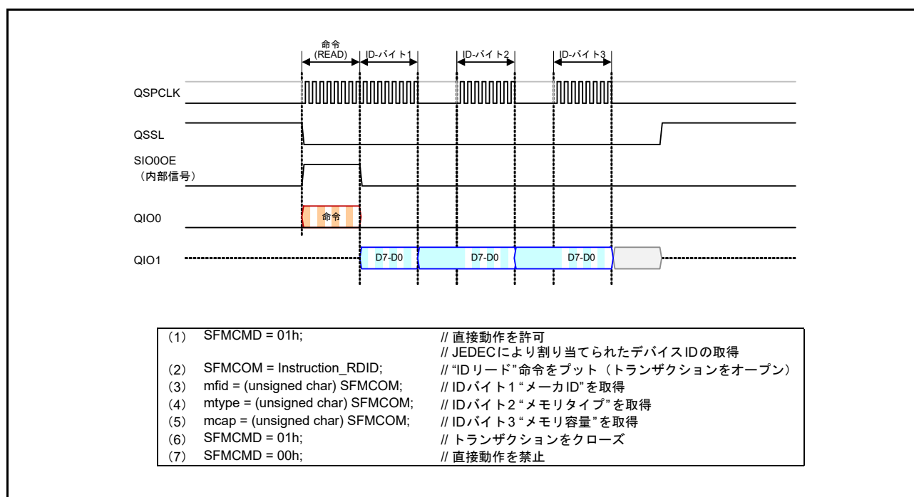
図 39.33 ID リードの直接通信タイミング例
