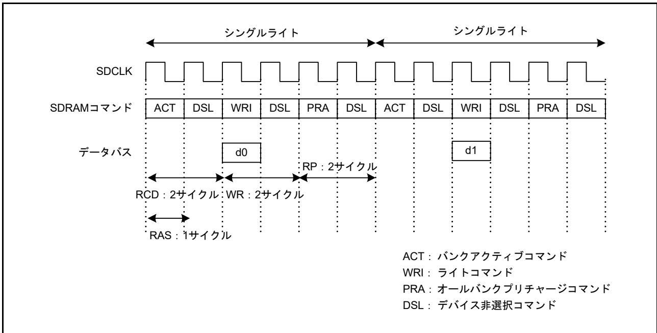
図 15.61 シングルライトタイミング例 (3)
