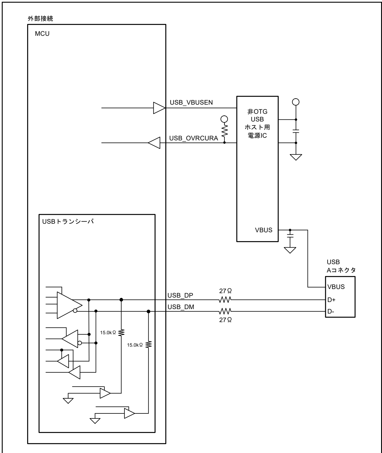
図 32.4 ホスト接続例
