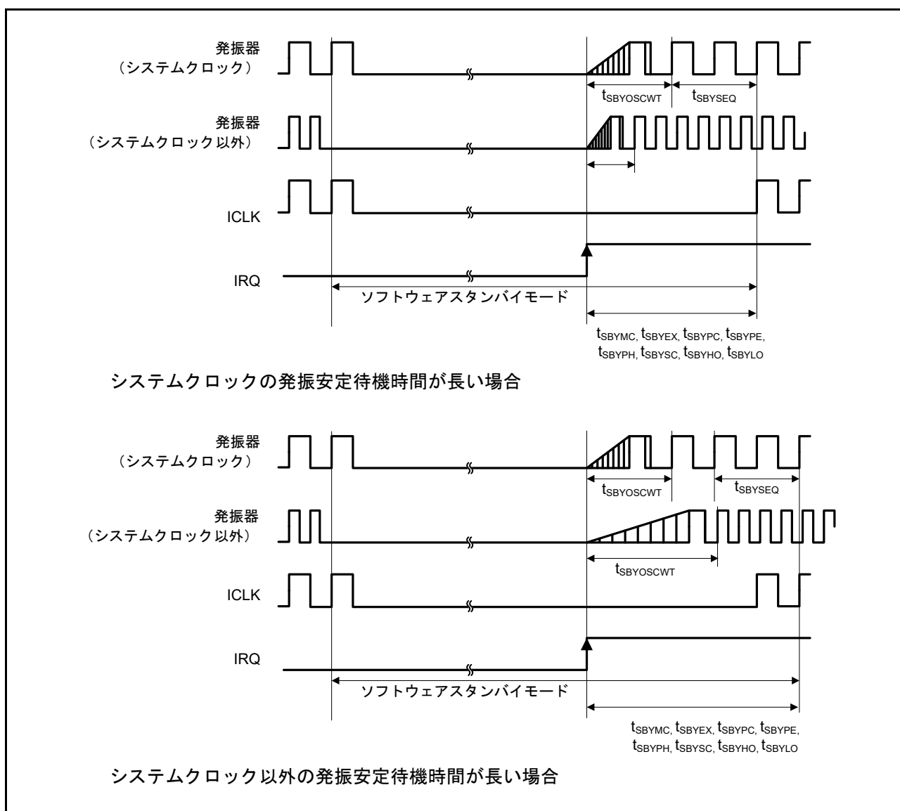
図 60.15 ソフトウェアスタンバイモード解除タイミング
