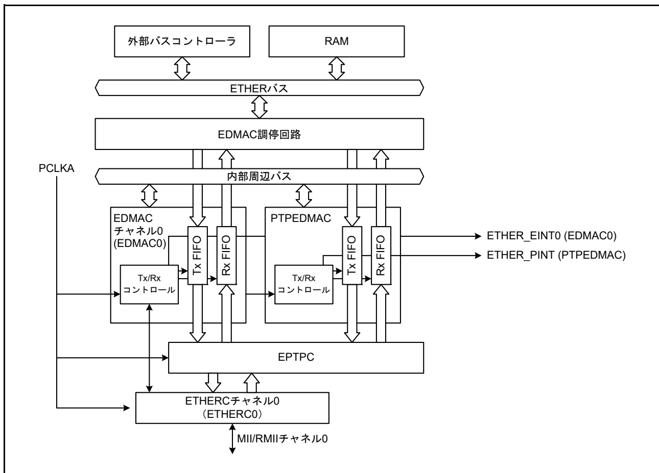
図 31.1 EDMAC の構成
