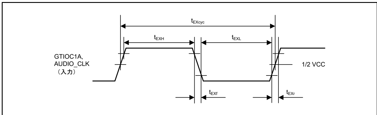
図 60.62 クロック入力タイミング
