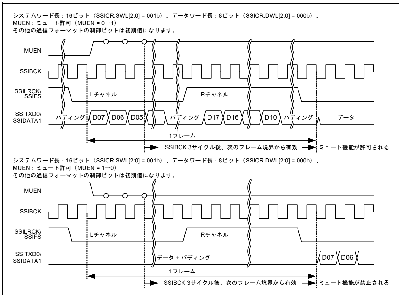
図 41.5 ミュート機能設定時の送信データ
