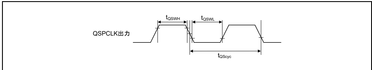
図 60.58 QSPI クロックタイミング
