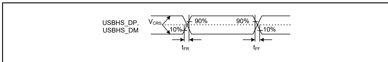
図 60.85 フルスピードモードにおける USBHS_DP、USBHS_DM の出力タイミング
