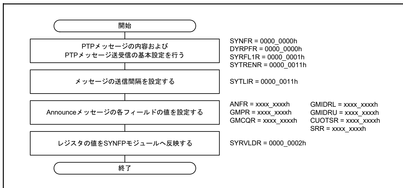
図 30.8 E2E マスタ動作の開始手順
