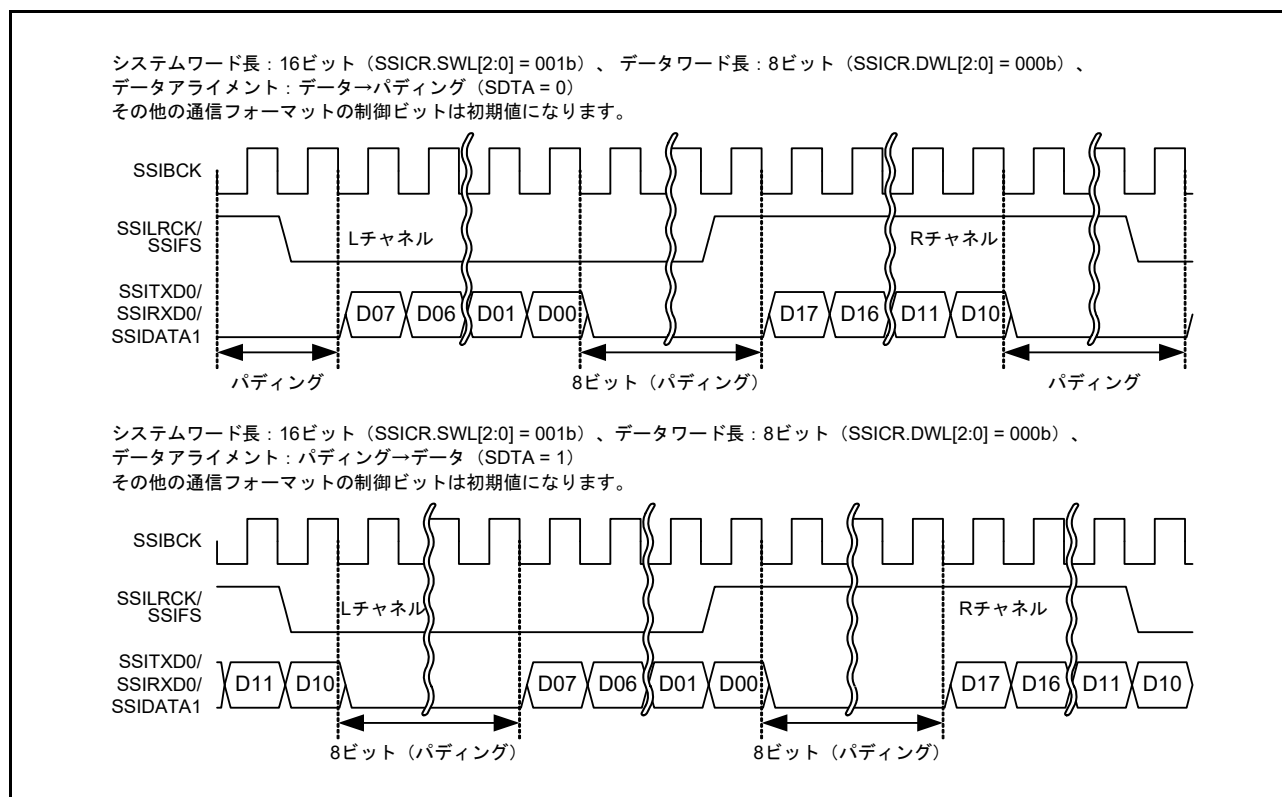
図 41.10 パディングビットのあるシリアルデータのアライメント設定
