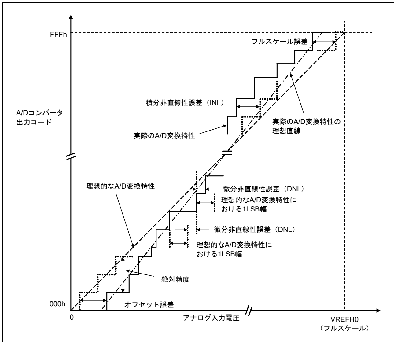
図 60.95 ADC12 特性用語の解説図
