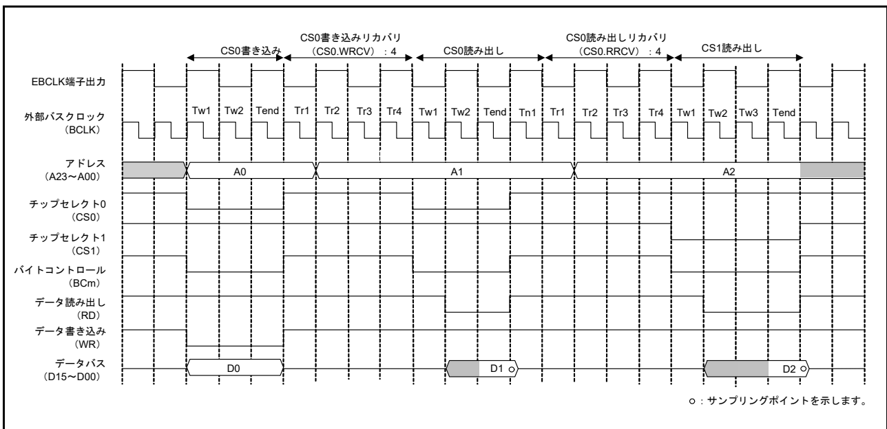
図 15.38 EBCLK 端子出力選択ビットで BCLK の 2 分周を選択した場合のリカバリサイクルの動作例（セパレートバスインタフェースによるノーマルアクセスの場合）（ m = 0, 1 ）
