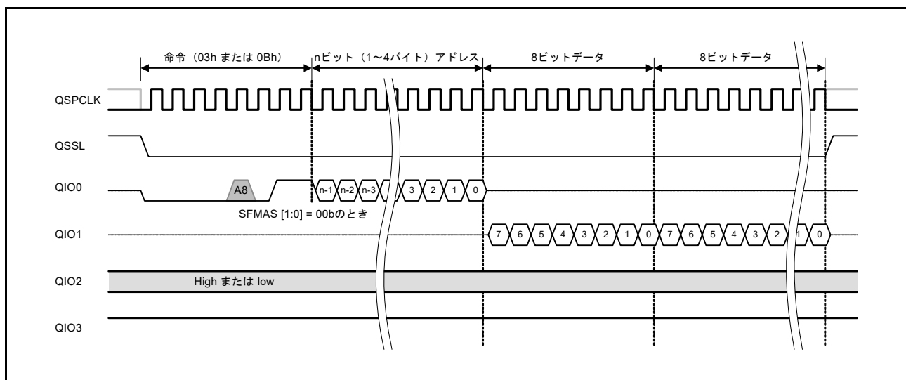
図 39.15 標準リードバスサイクル
