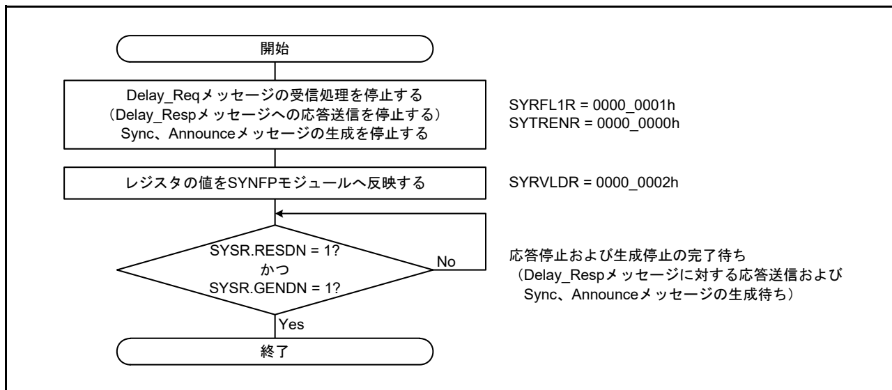
図 30.10 E2E マスタ動作の停止手順
