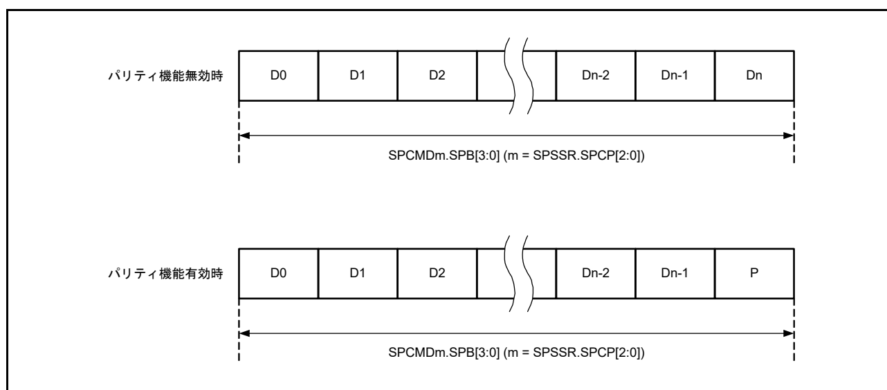
図 38.13 パリティ機能無効時と有効時のデータフォーマット
