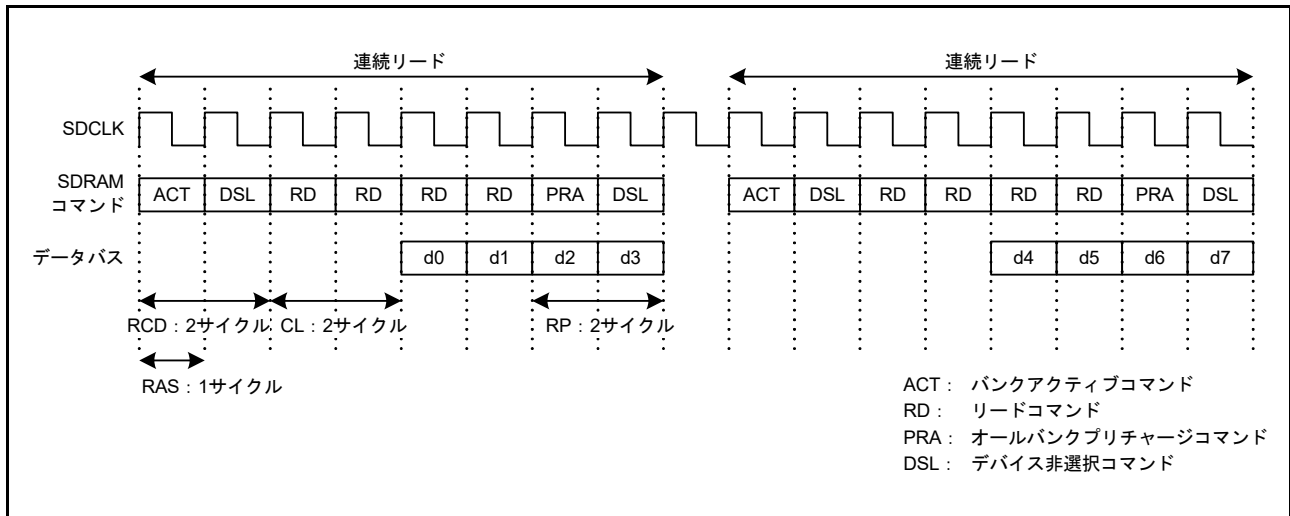
図 15.65 連続リードタイミング例 (2)
