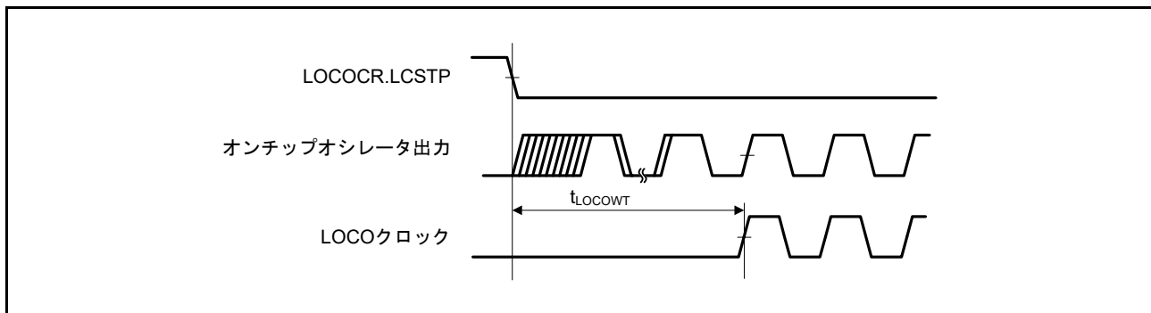
図 60.10 LOCO クロック発振開始タイミング
