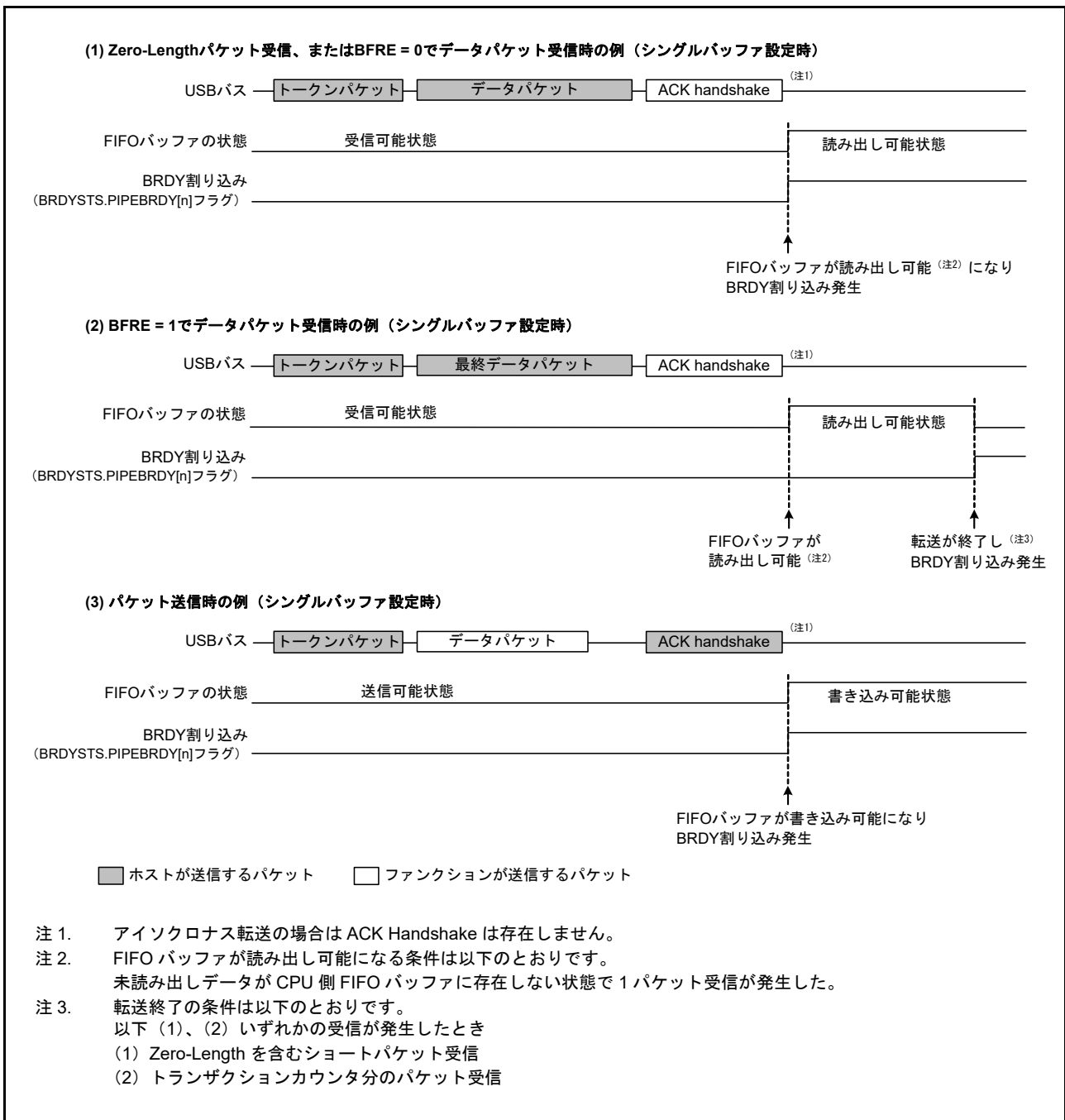
図 33.5 BRDY 割り込み発生タイミング
