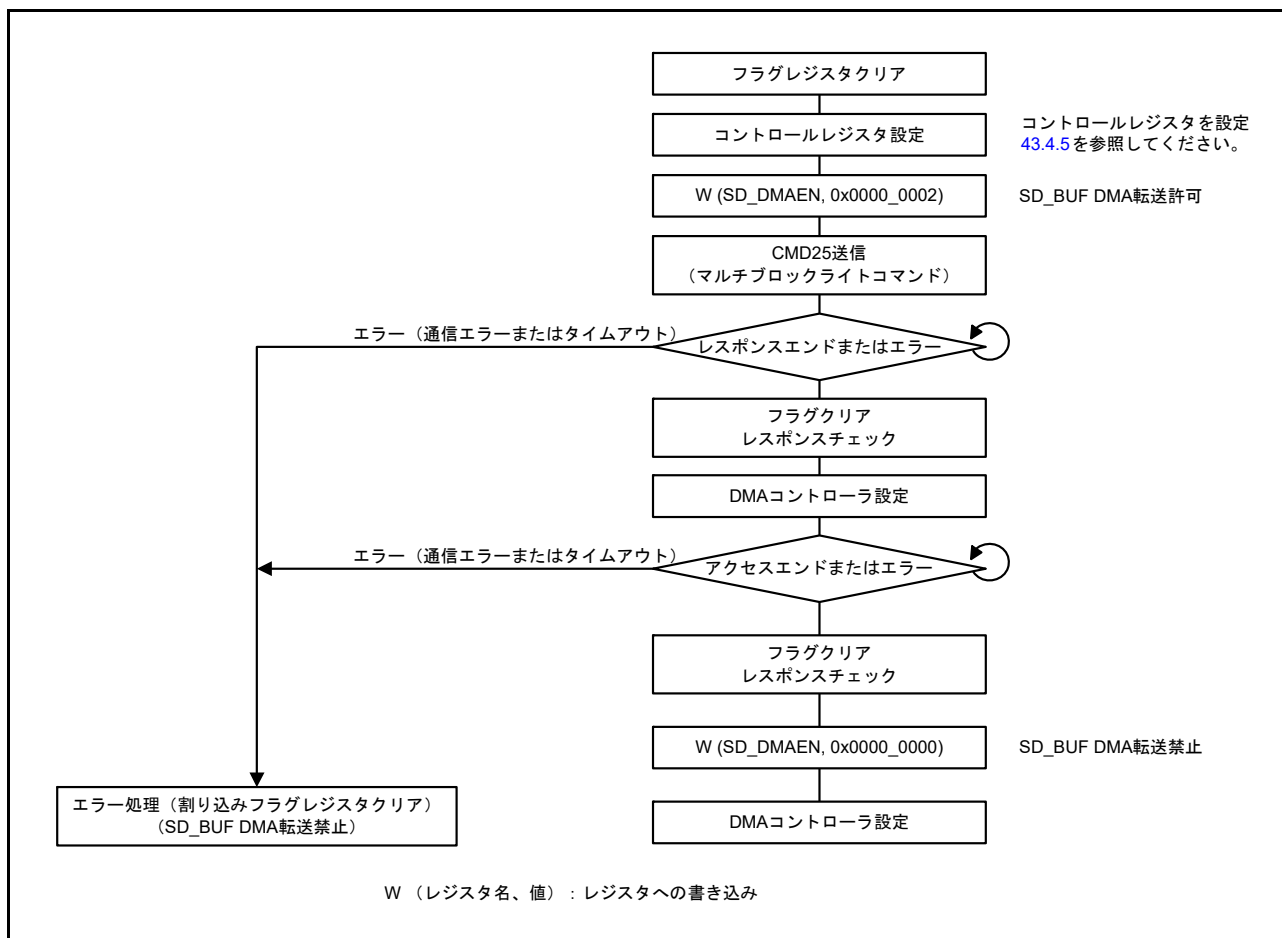
図 43.24 SD_BUF_DMA ライト動作の例
