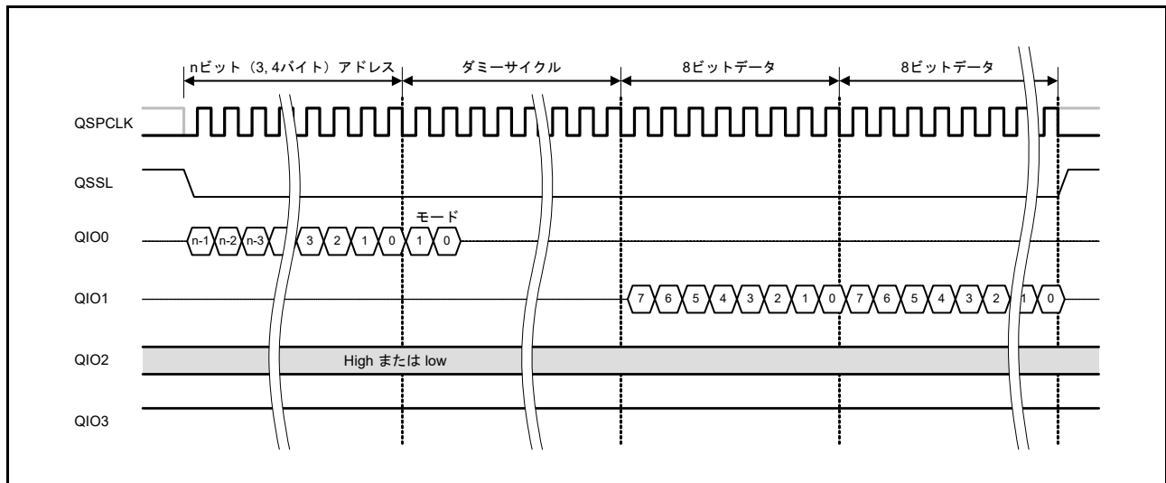
図 39.17 XIP モード時のファストリードバスサイクル
