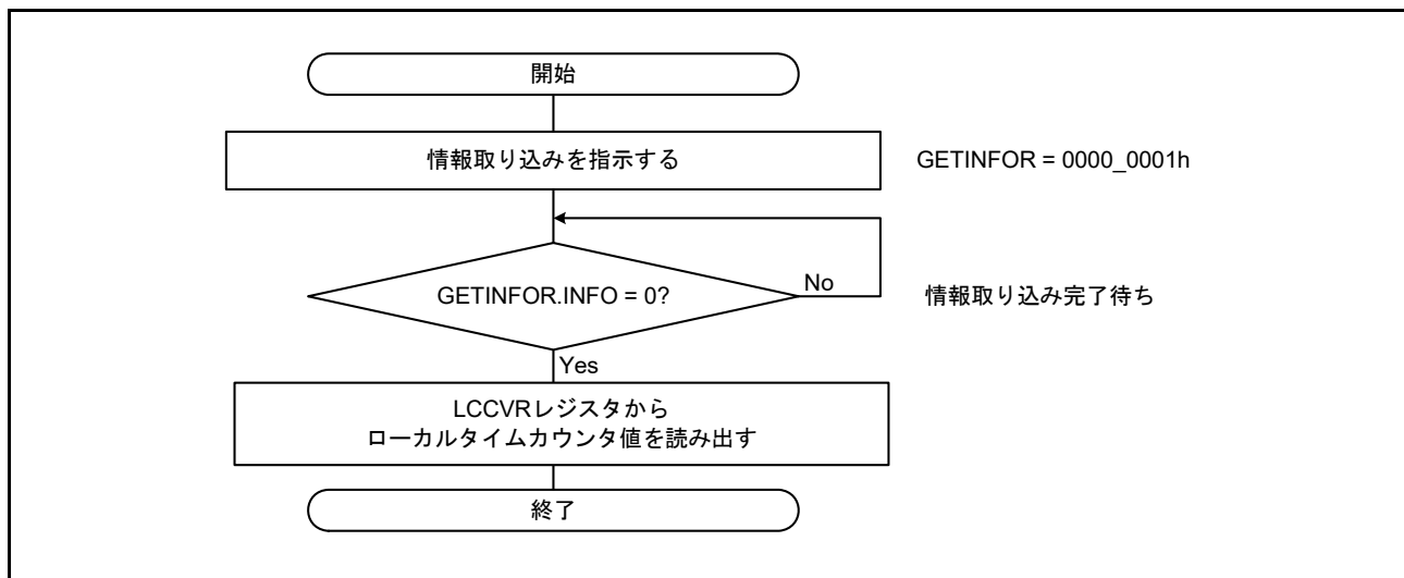
図 30.27 ローカルクロックカウンタからの時刻の読み出し手順
