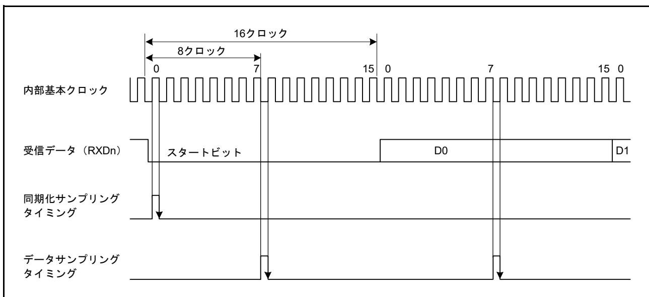
図 34.3 調歩同期式モードでの受信データのサンプリングタイミング
