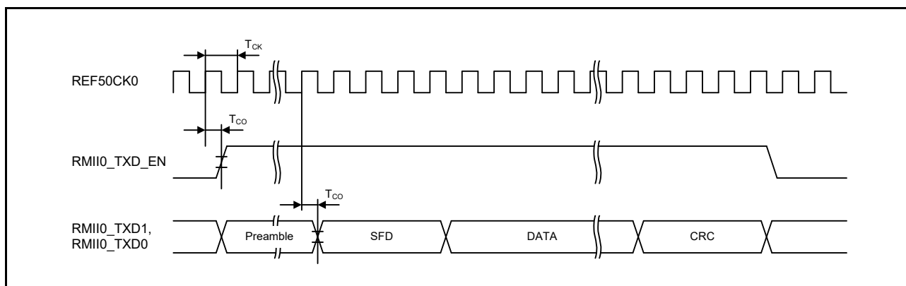
図 60.68 RMII 送信タイミング
