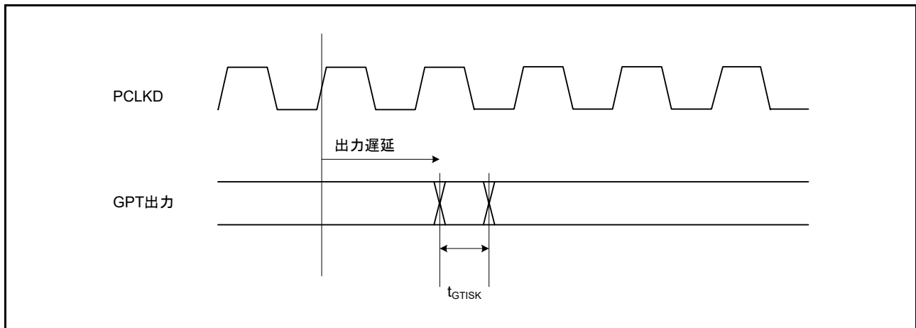
図 60.37 GPT 出力遅延スキュー
