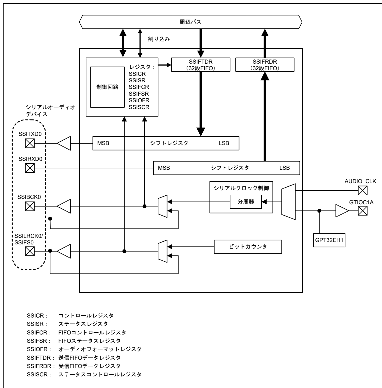
図 41.2 SSIE ブロック図 (SSIE0)
