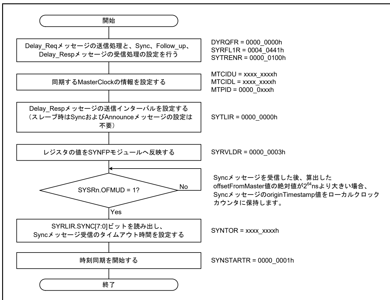
図 30.11 E2E スレーブ動作の開始手順
