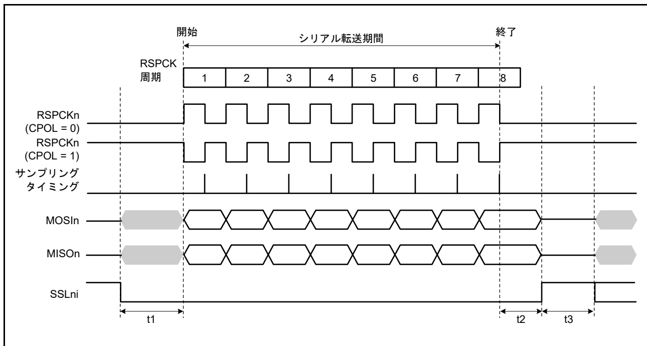
図 38.23 SPI 転送フォーマット (CPHA ビット = 1)
