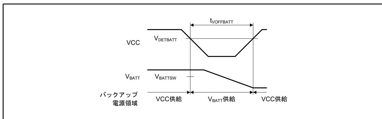
図 60.101 バッテリバックアップ機能特性
