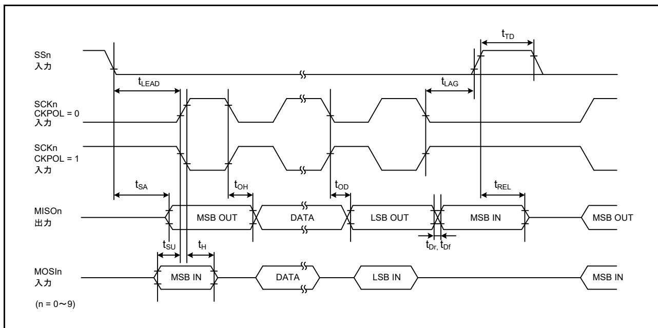
図 60.48 CKPH = 1 の場合におけるスレーブの SCI 簡易 SPI モードタイミング
