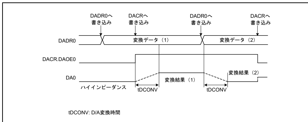
図 48.2 DAC12の動作例
