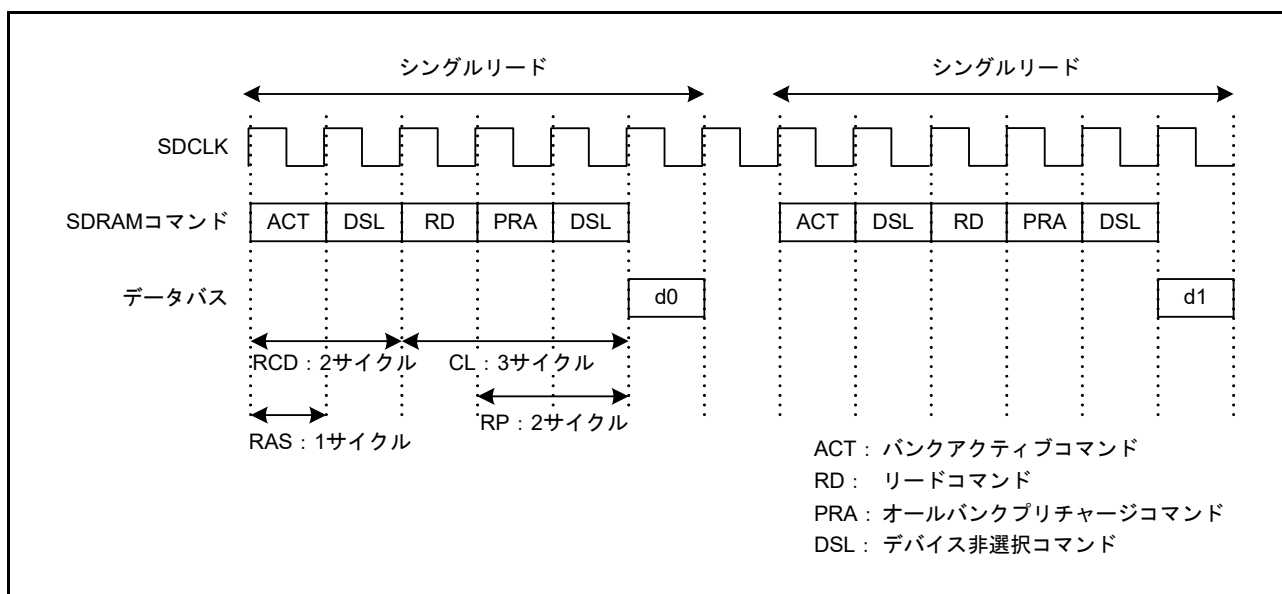
図 15.56 シングルリードタイミング例 (3)
