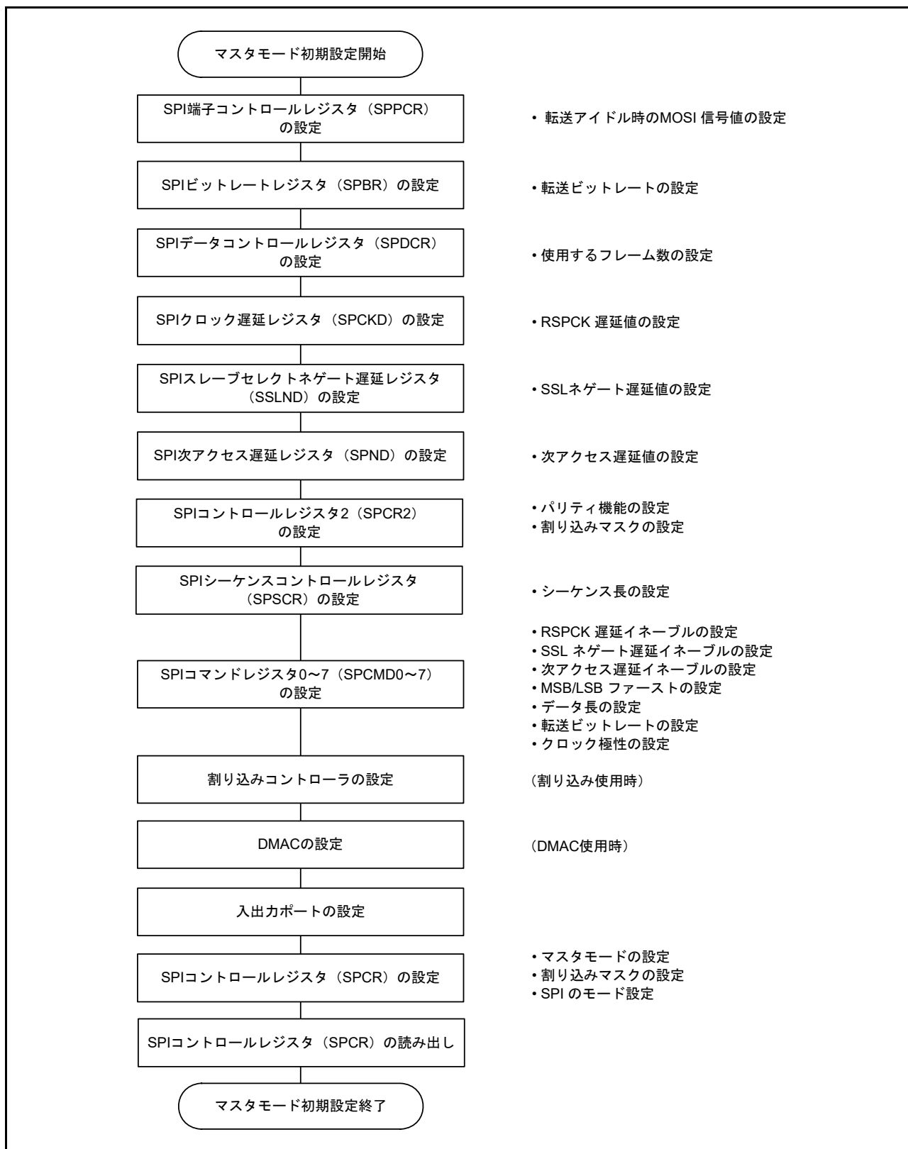
図 38.47 マスタモード時のクロック同期式動作の初期化フロー例
