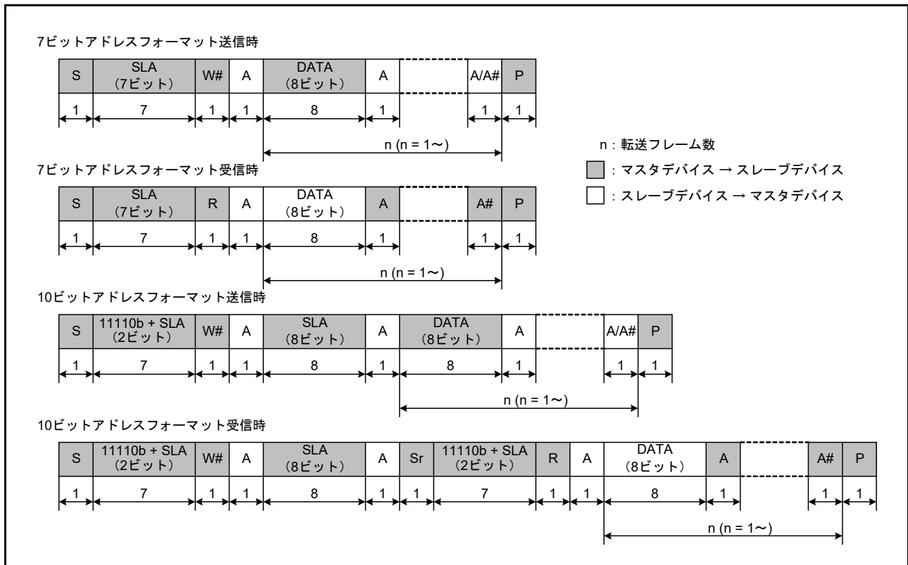
図 34.58 I 2 C バスフォーマット
