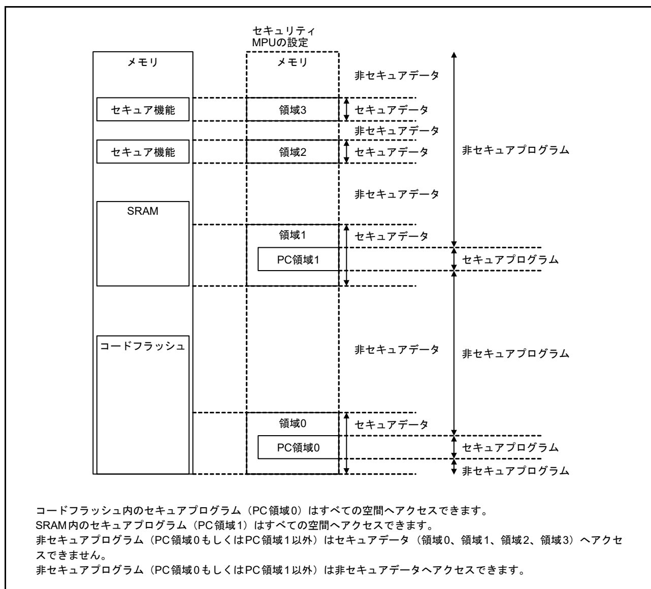
図 16.11 セキュリティ MPU の使用例
