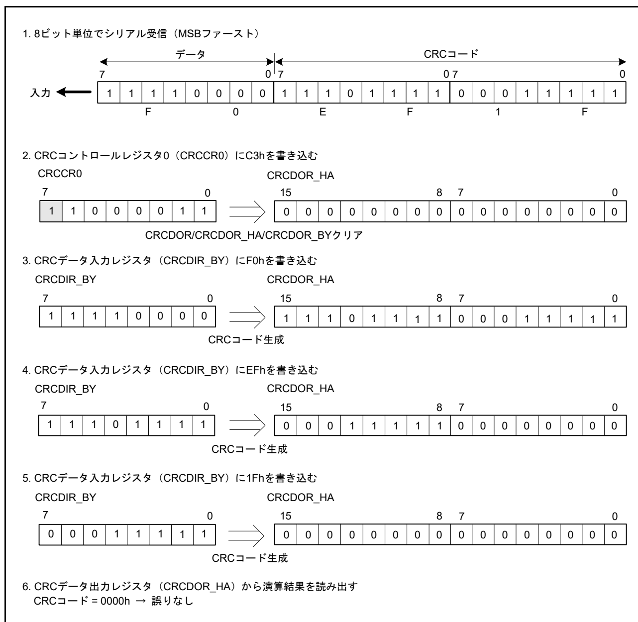
図 40.5 MSB ファーストのデータ受信
