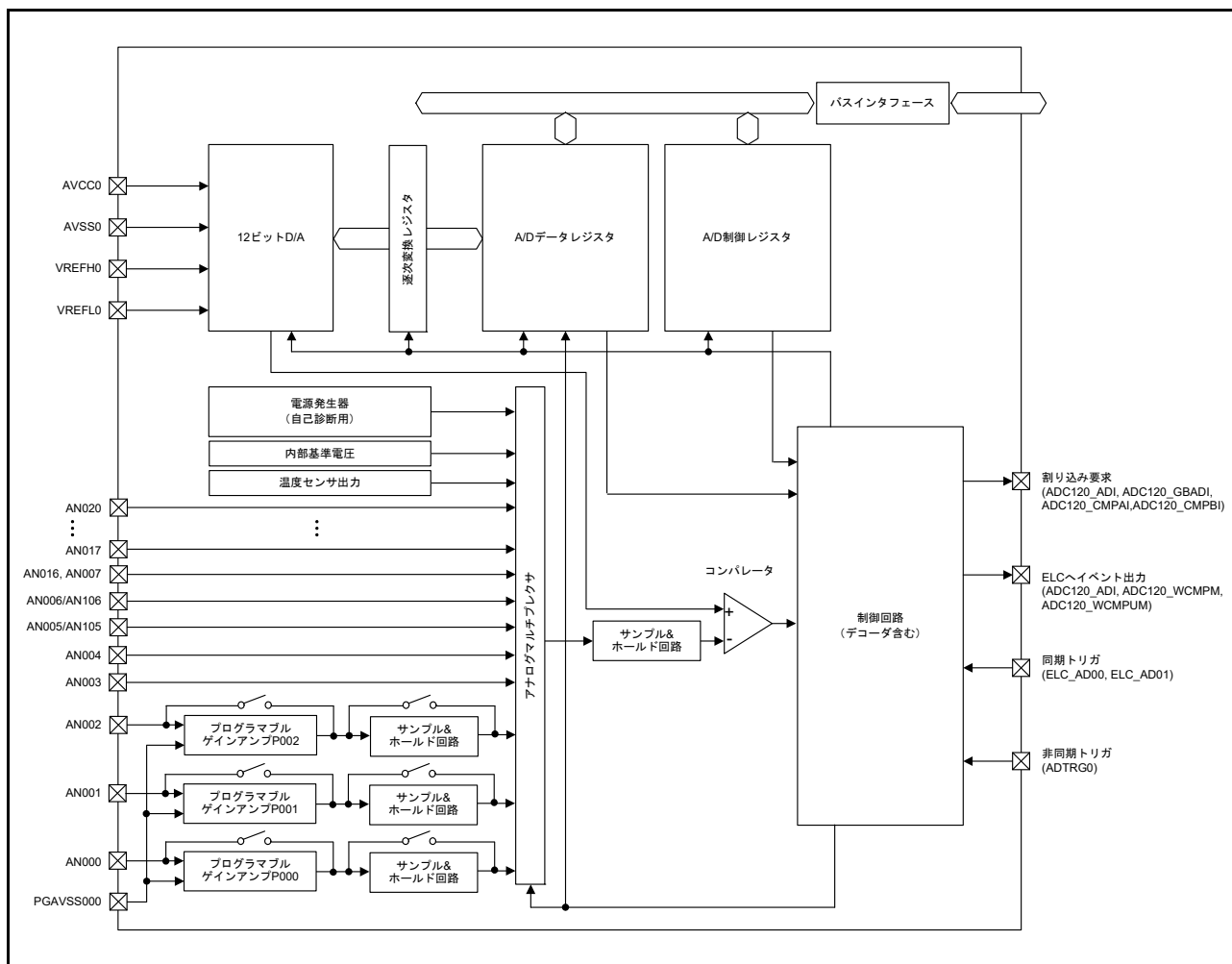
図 47.1 ADC12 (ユニット0) のブロック図
