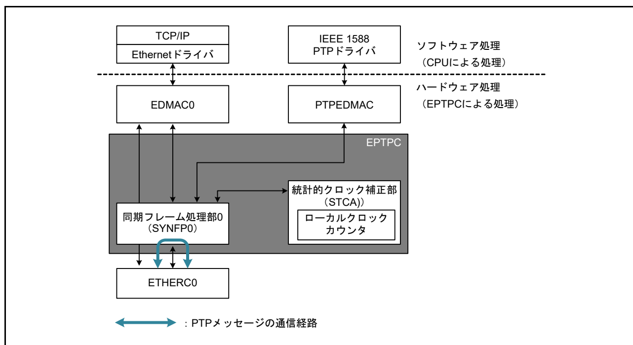
図 30.6 ハードウェアによる PTP メッセージの生成と応答の経路
