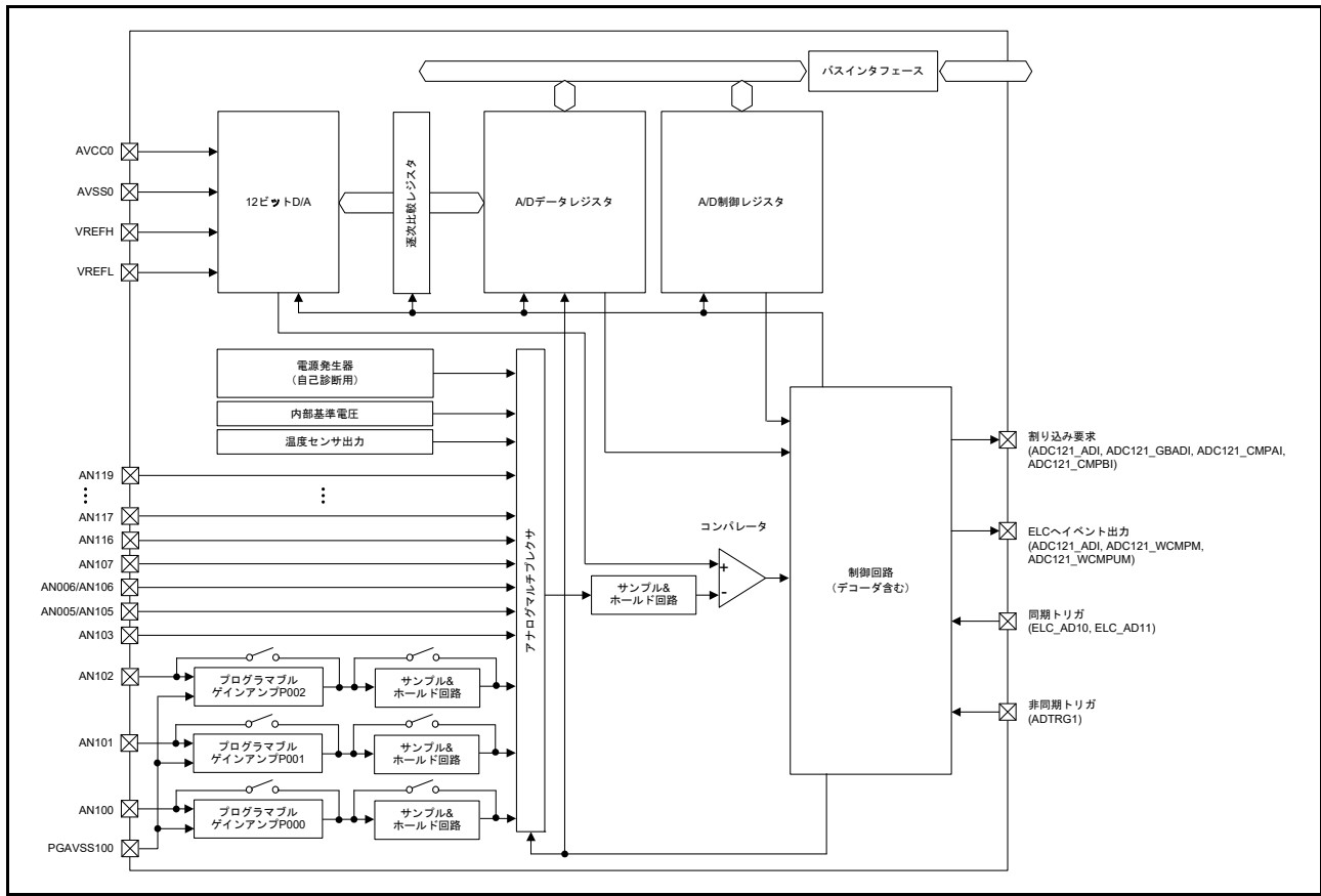
図 47.2 ADC12 (ユニット1) のブロック図
