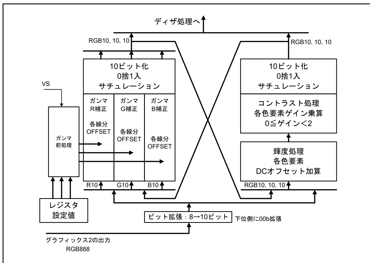
図 58.6 パネル用補正回路の構成
