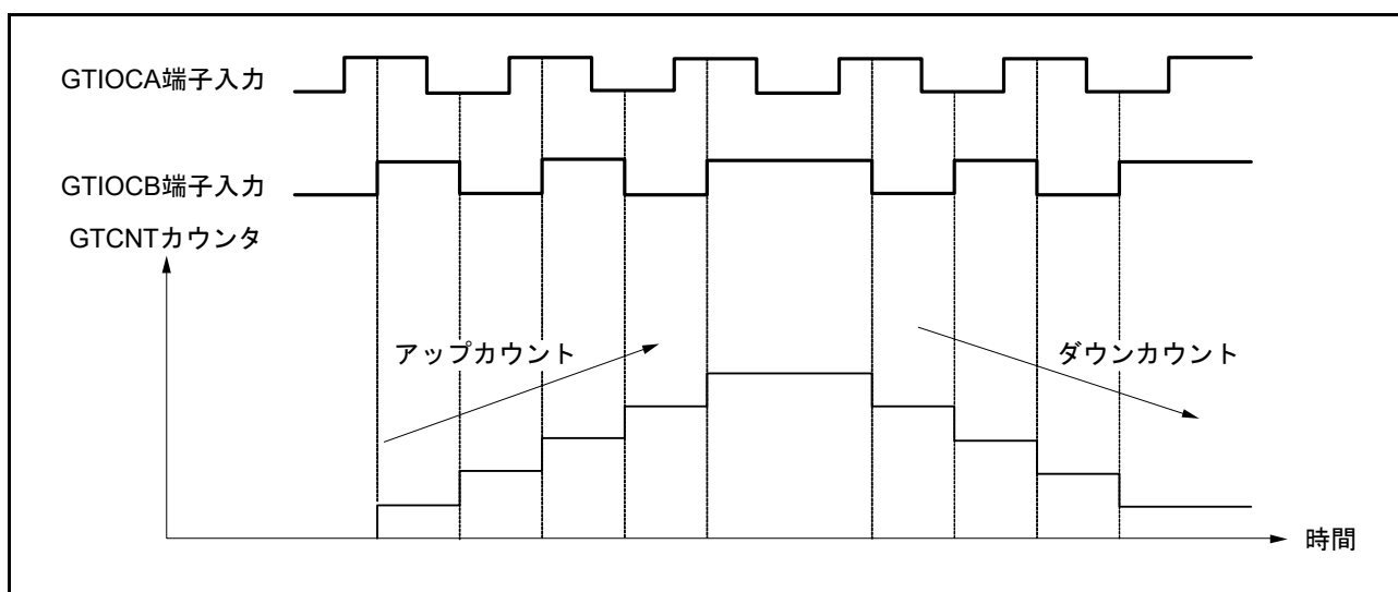
図 23.78 位相計数モード4の動作例
