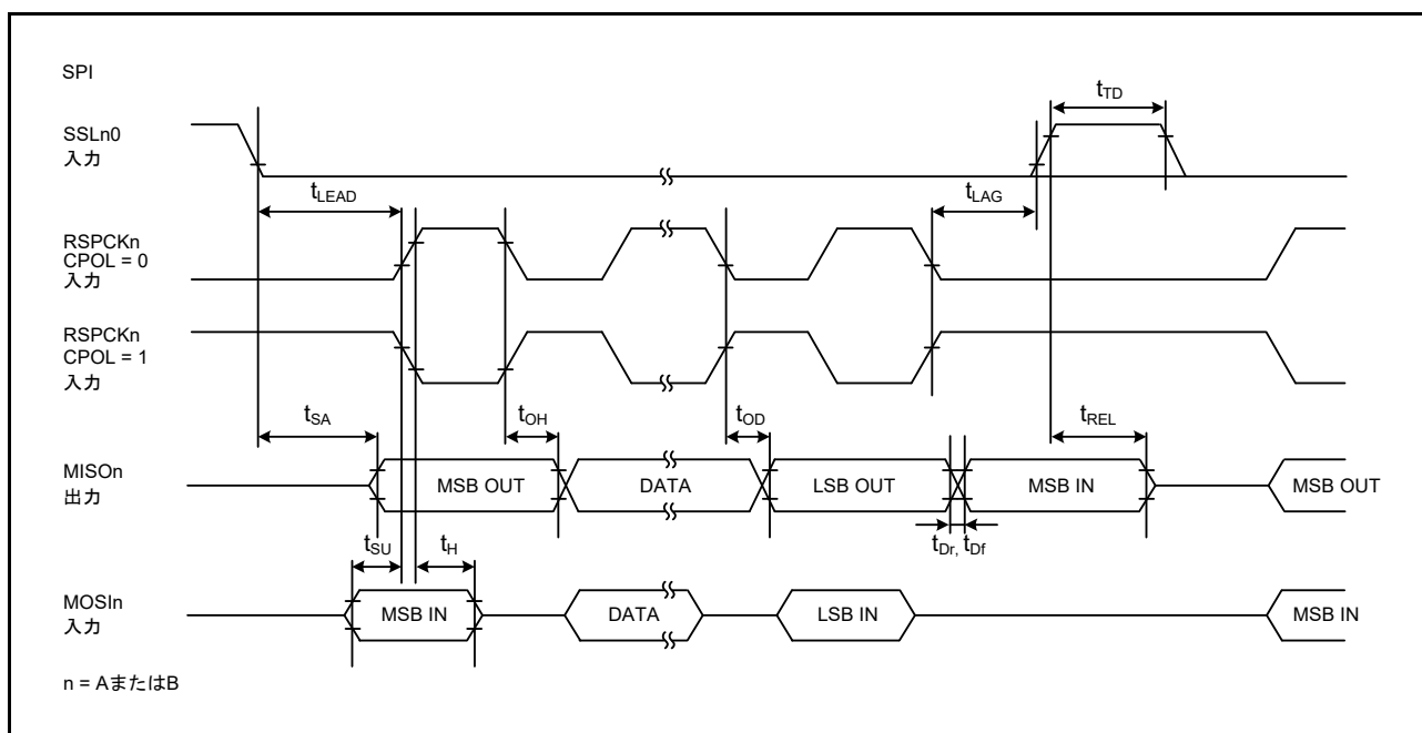
図 60.56 CPHA = 0 の場合におけるスレーブの SPI タイミング
