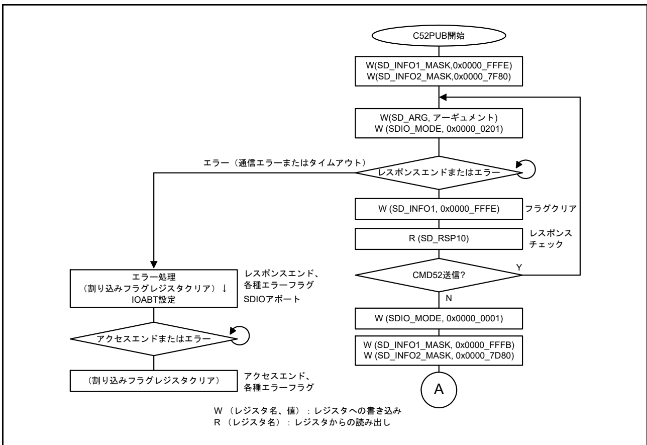
図 43.22 CMD53 マルチブロックライト時に CMD52 (SDIO none abort) が送信される場合のフロー
