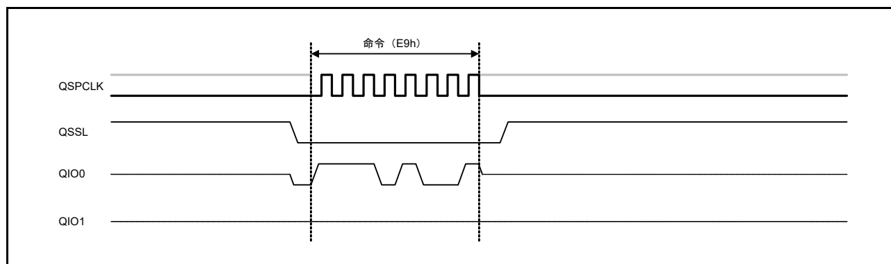
図 39.27 4バイトモード解除バスサイクル
