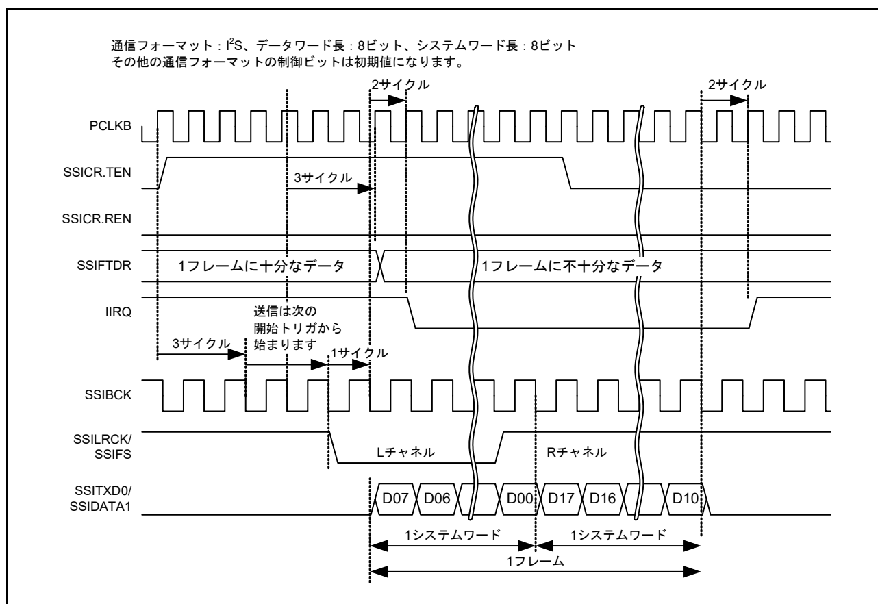
図 41.14 IIRQ 設定タイミング (送信)
