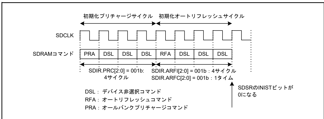
図 15.49 SDRAM 初期化シーケンスのタイミング例
