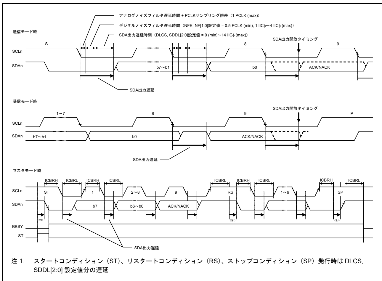
図 36.22 SDA出力遅延機能
