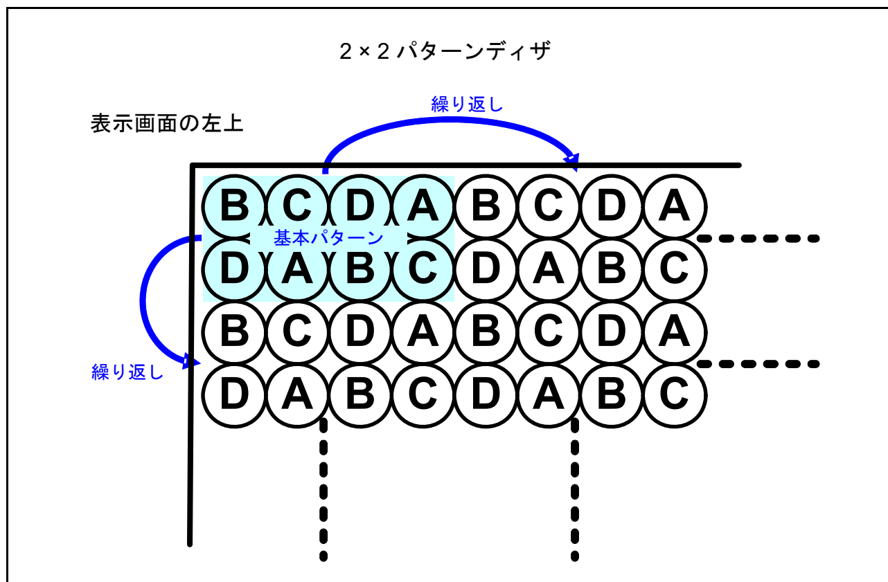
図 58.14 2x2 パターンディザの追加値選択方法
