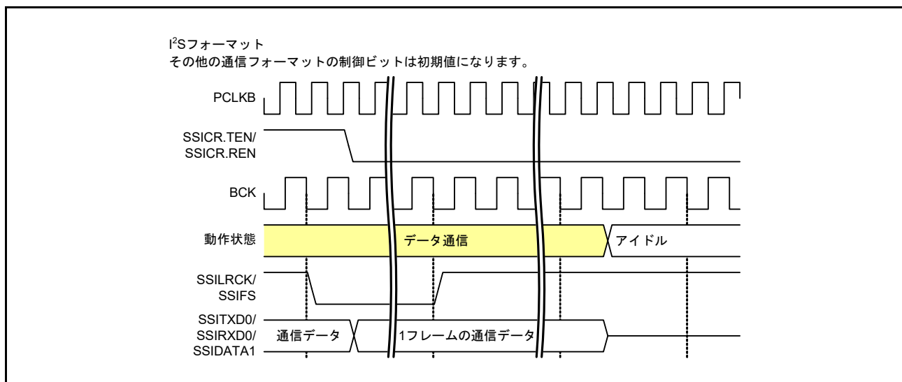
図 41.48 データ通信からの停止 (パディングビットなし)
