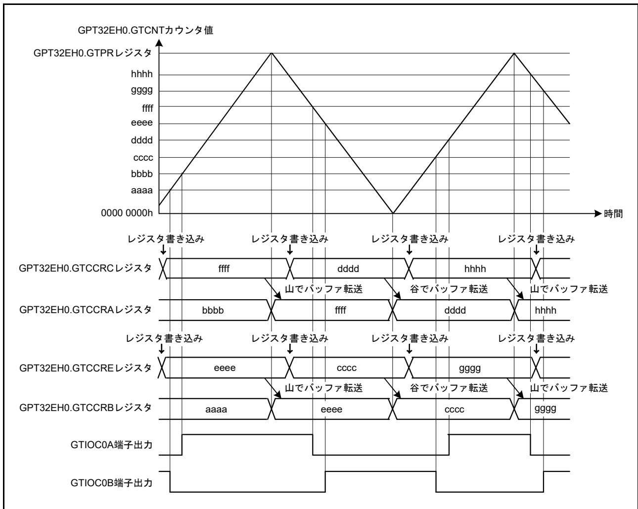
図 23.39 三角波 PWM モード 2 動作例 (バッファ動作、カウントスタート時 GTIOC0A 端子 = Low 出力 / GTIOC0B 端子 = High 出力、GTCCRA/GTCCRB レジスタのコンペアマッチでトグル出力、周期の終わりで出力保持の場合)
