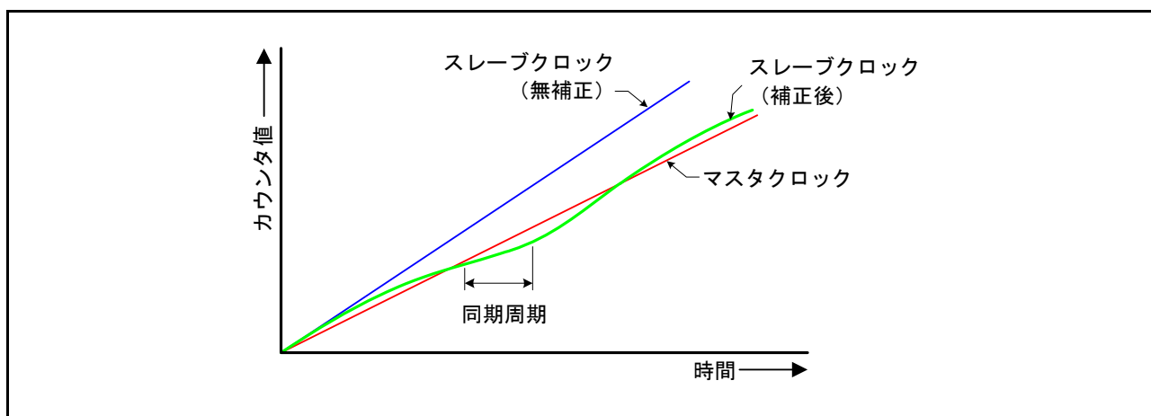
図 30.21 時刻補正の概念
