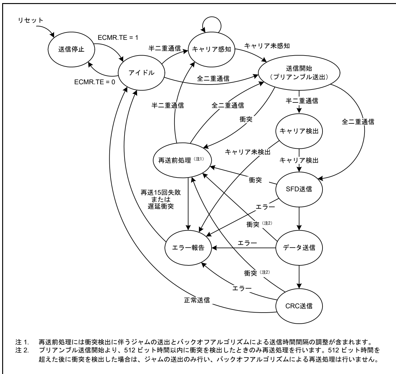
図 29.4 ETHERC 送信部状態遷移図
