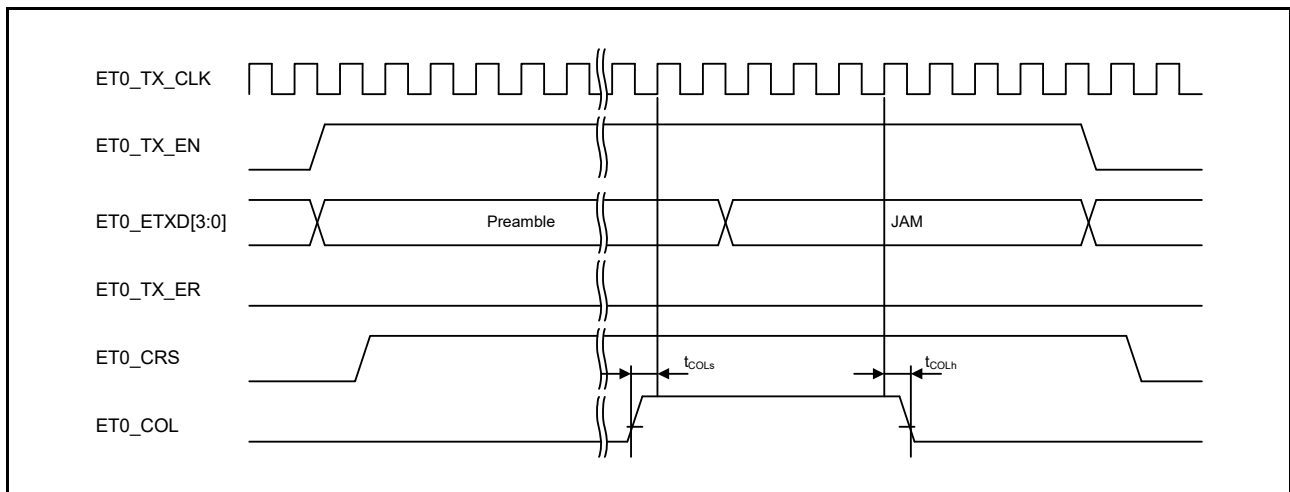
図 60.73 競合発生時の MII 送信タイミング
