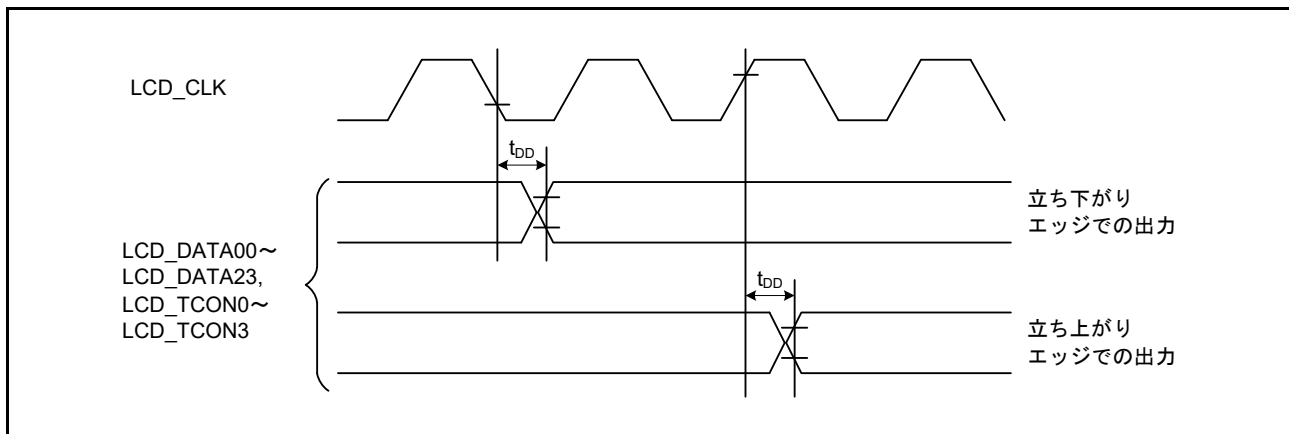
図 60.82 表示出力タイミング
