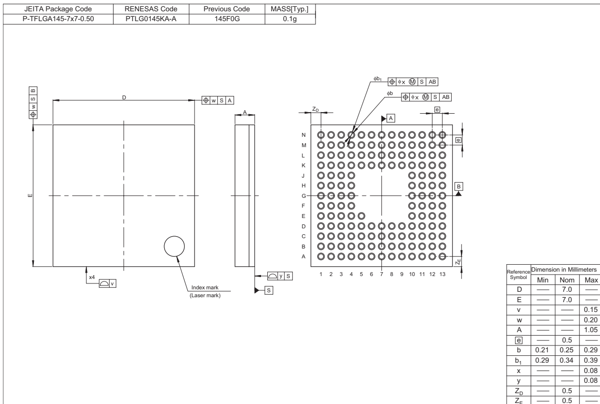
図 2.3 145-pin LGA
