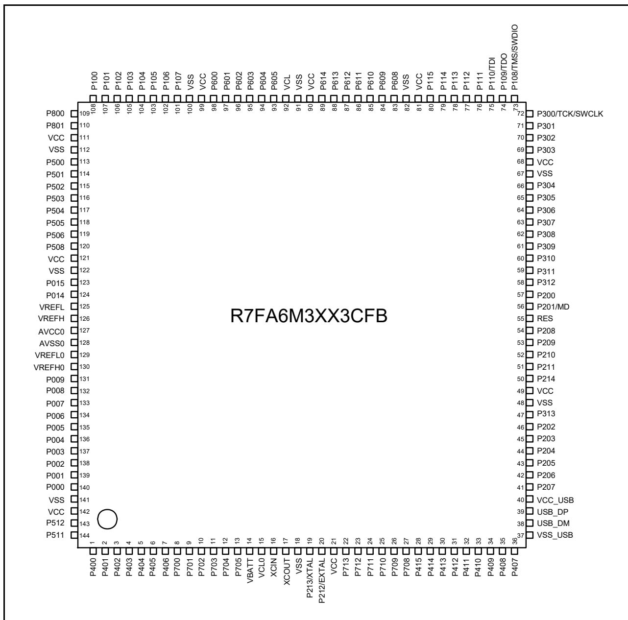
図 1.6 144-pin LQFP のピン配置図 (上面図)
