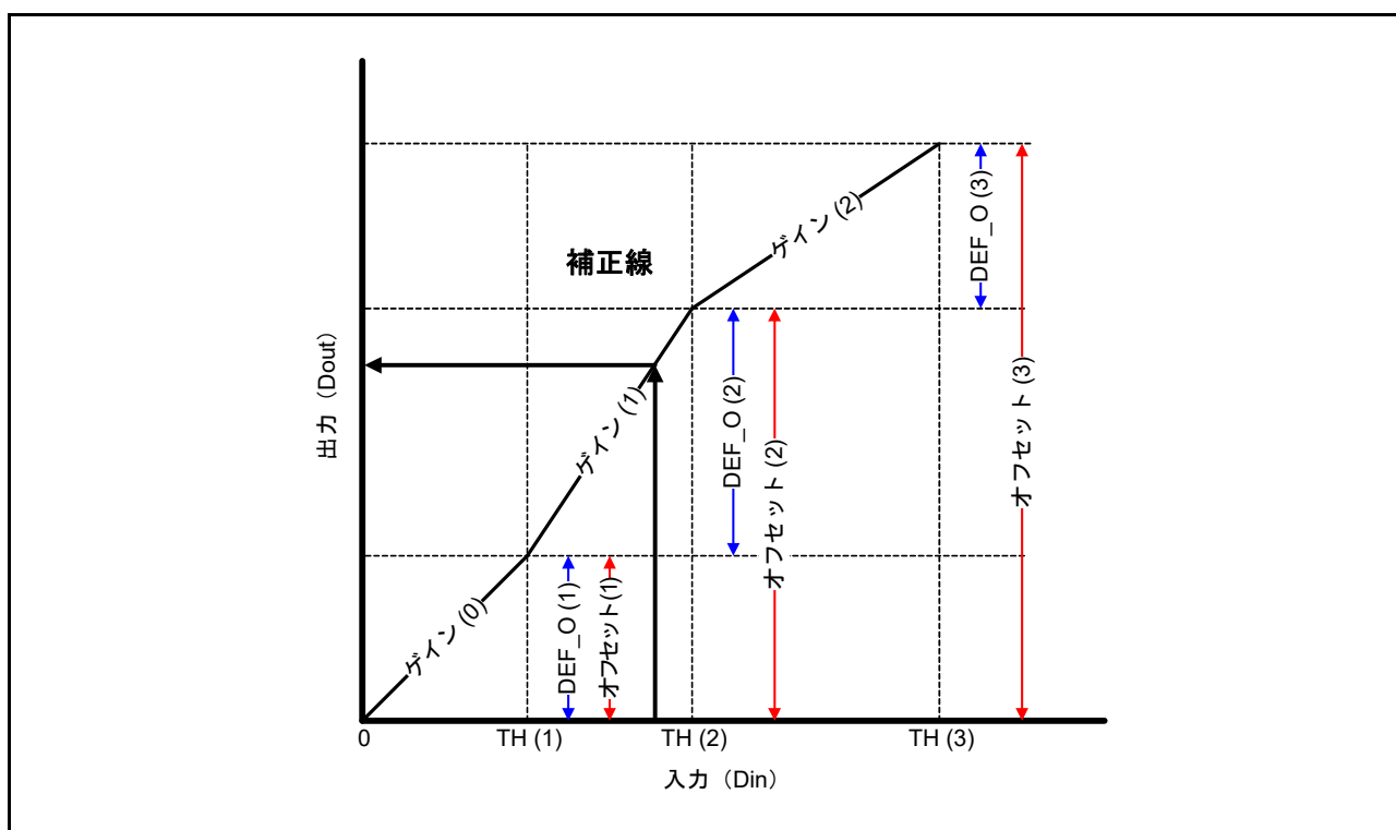
図 58.12 ガンマ補正値の計算
