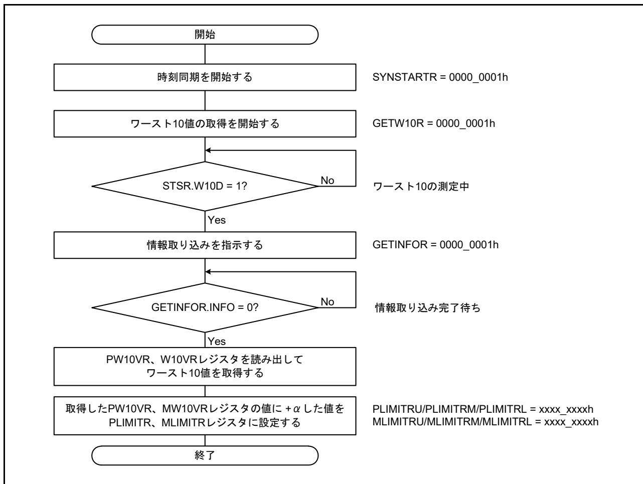
図 30.25 ソフトウェアによるワースト 10 値取得手順例
