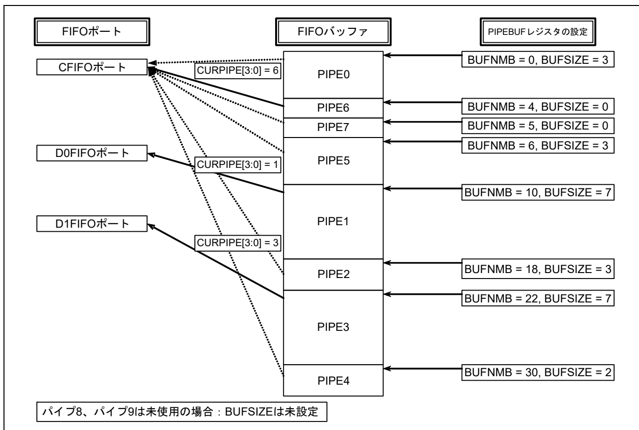
図 33.11 FIFO バッファのメモリマップ例
