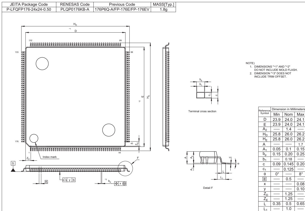
図 2.2 176-pin LQFP
