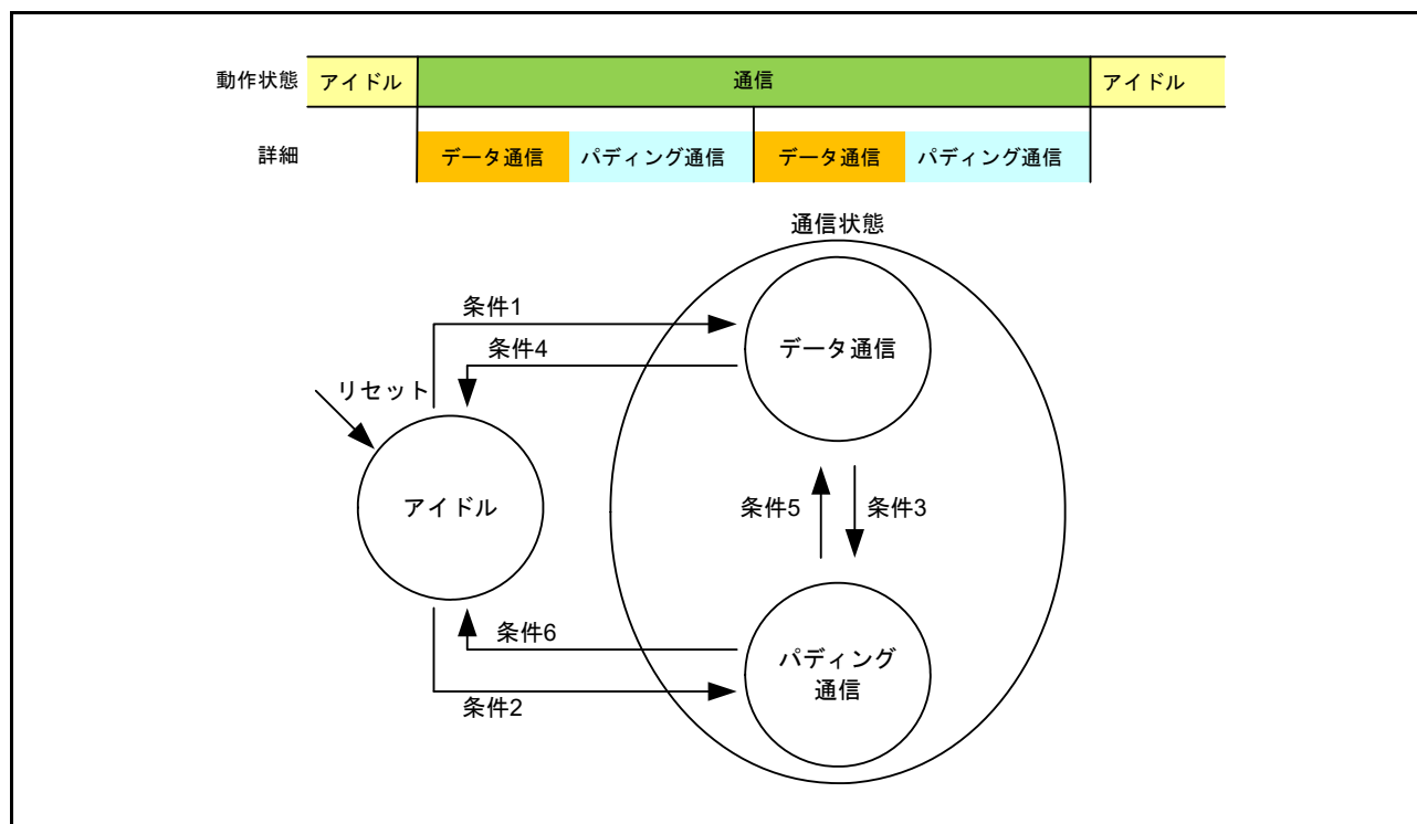
図 41.46 通信の状態遷移
