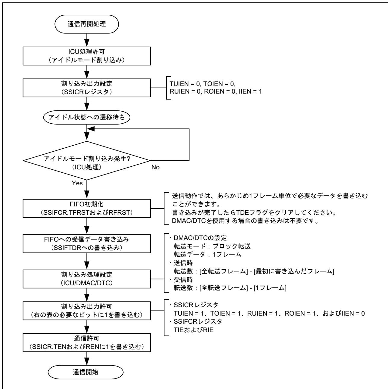
図 41.58 通信再開手順 (CPU 動作手順)
