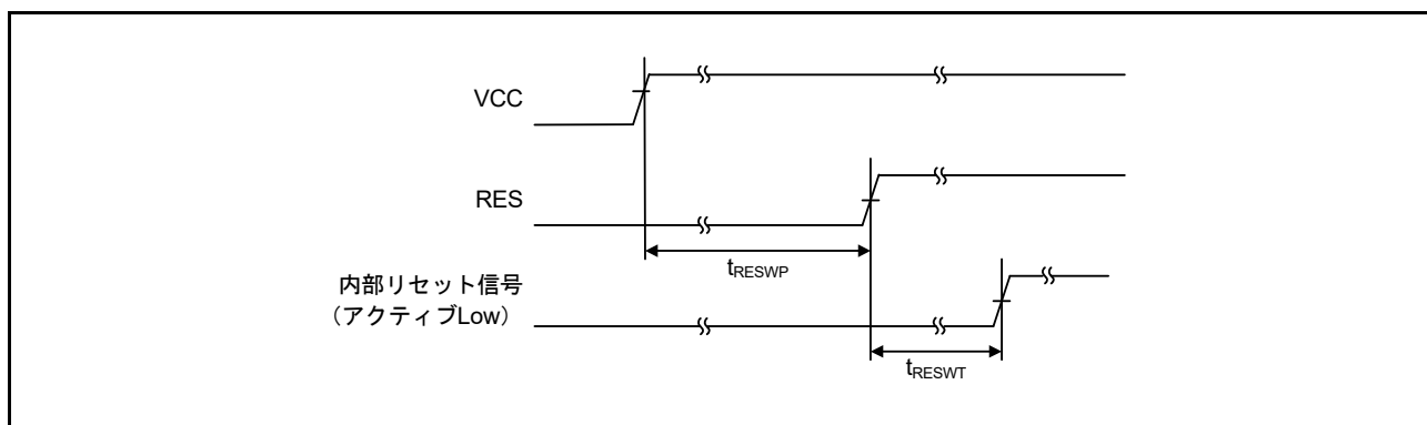
図 60.13 パワーオンリセットタイミング
