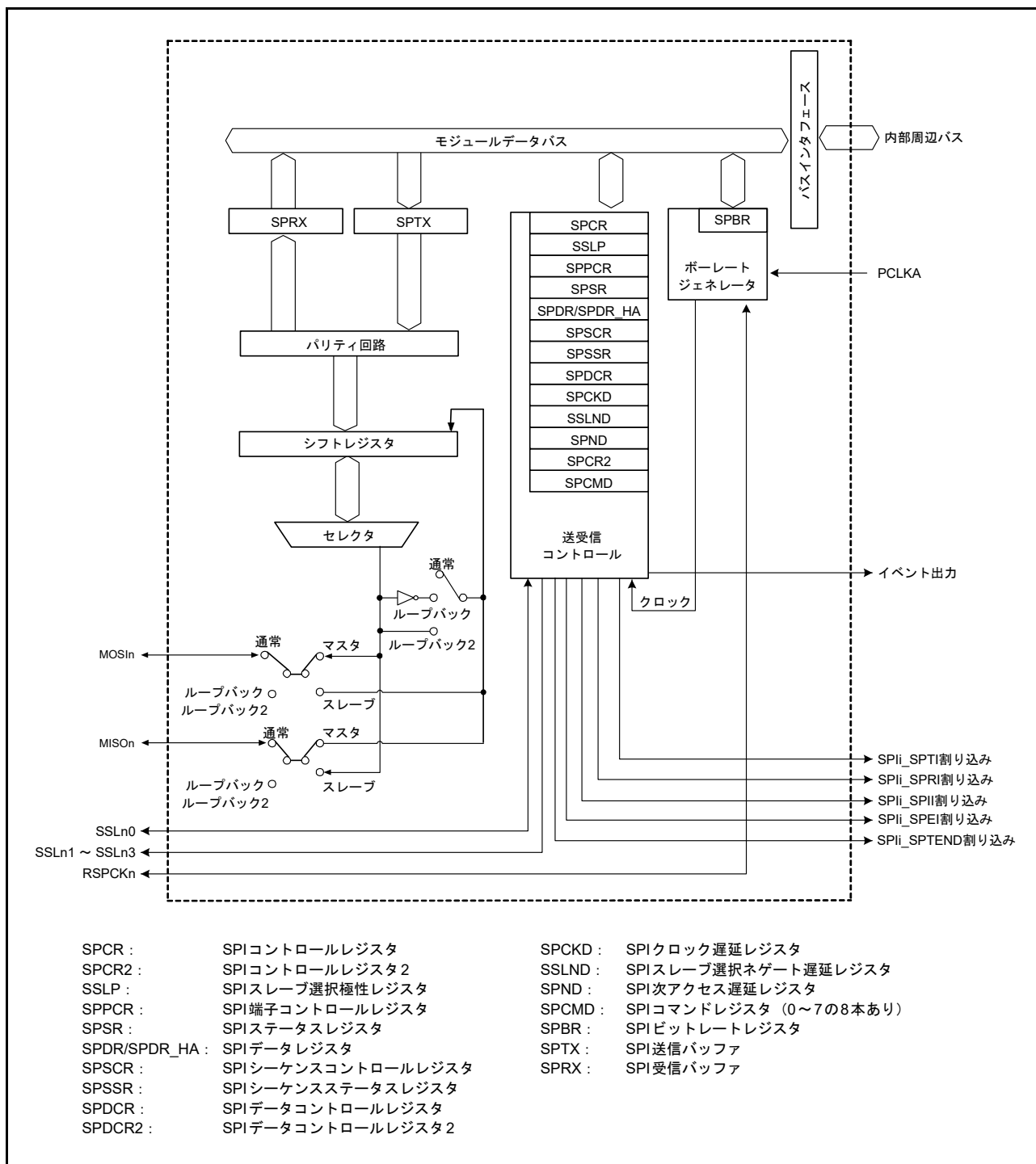
図 38.1 SPIのブロック図
