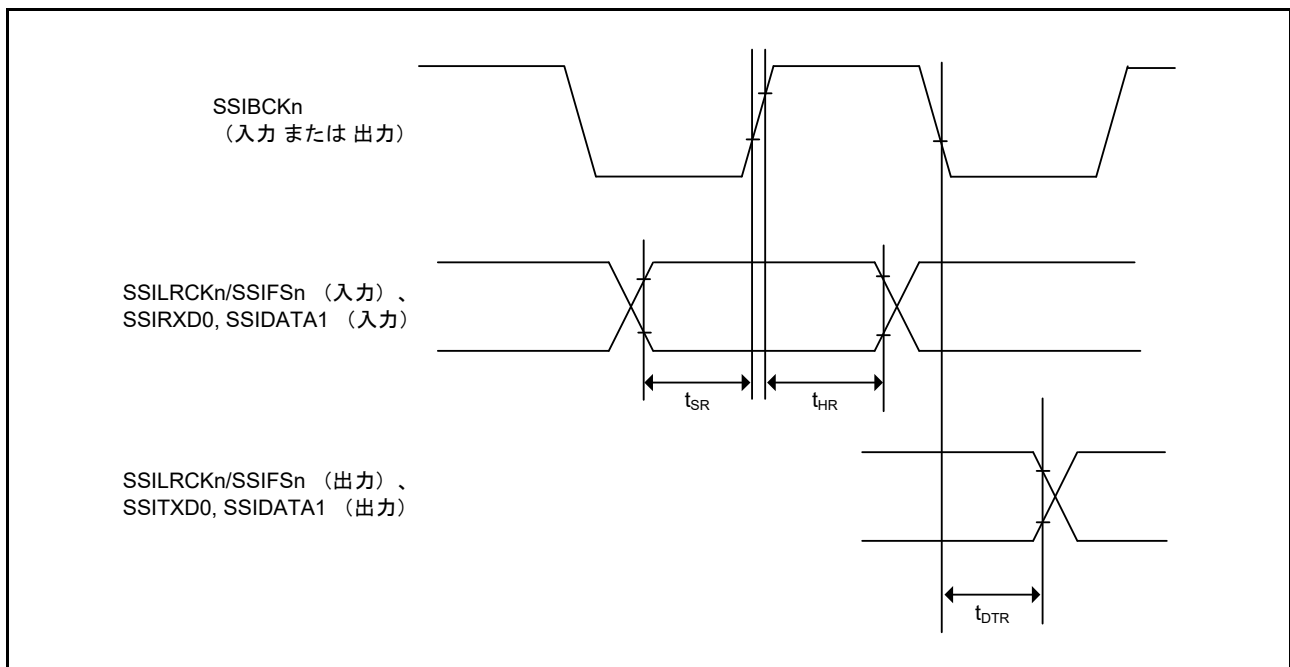
図 60.63 SSICR.BCKP = 0 の場合の SSIE データ送受信タイミング
