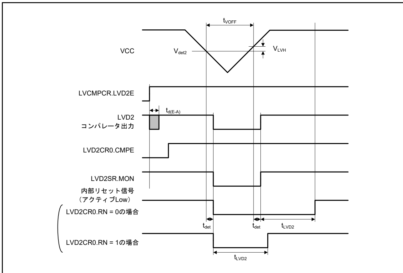
図 60.100 電圧検出回路タイミング ( V_{det2} )
