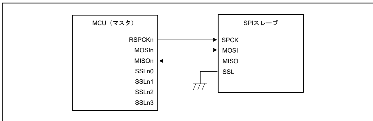
図 38.5 シングルマスタおよびシングルスレーブの構成例 (MCU はマスタ)
