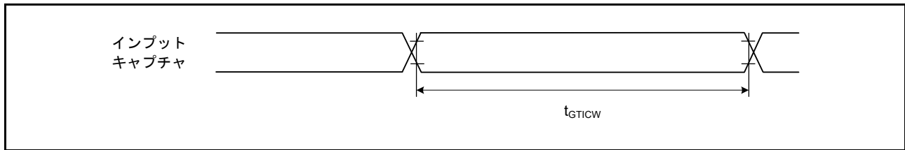
図 60.36 GPT インพุットキャプチャタイミング
