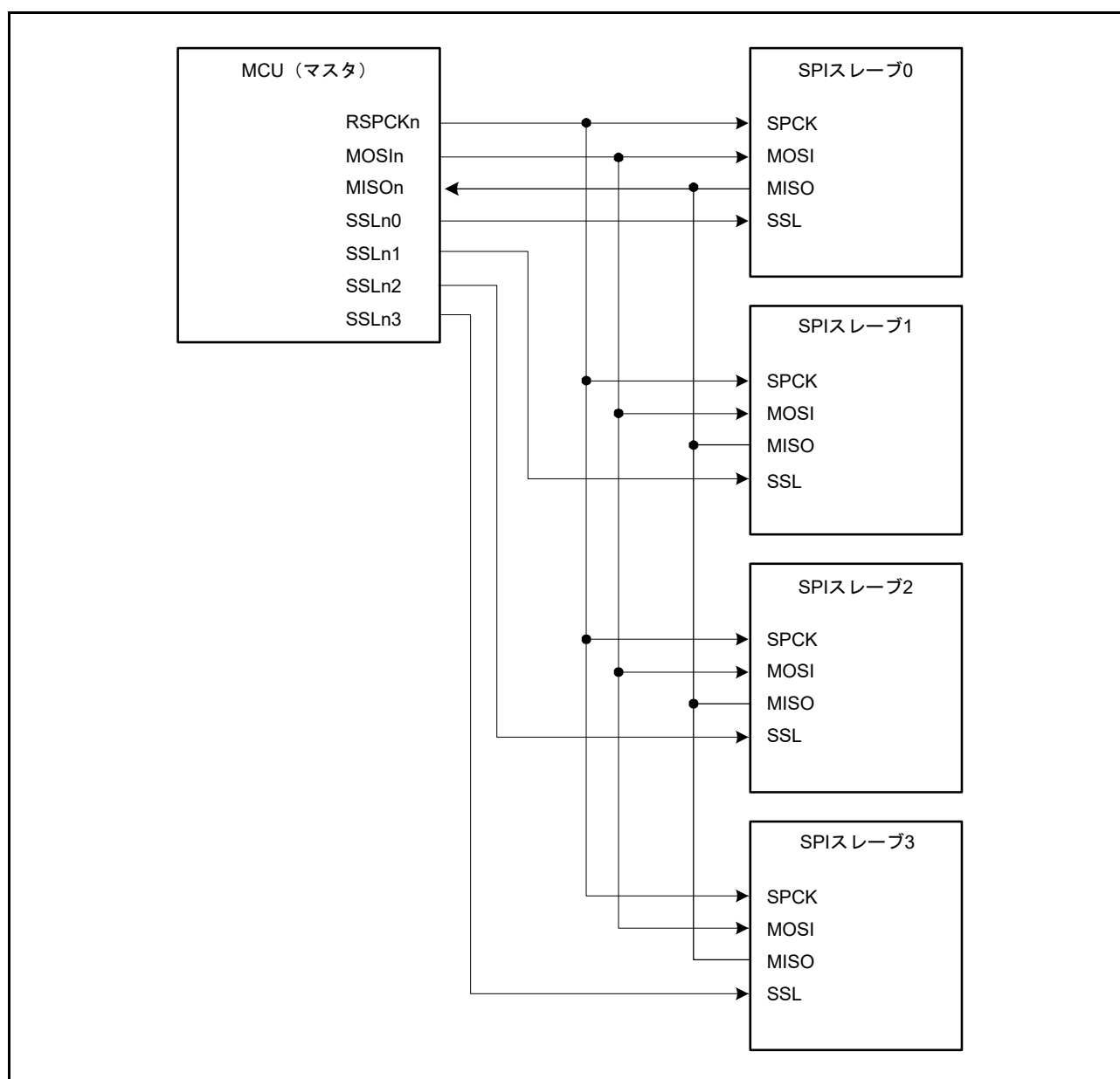
図 38.8 シングルマスタおよびマルチスレーブの構成例 (MCU はマスタ)
