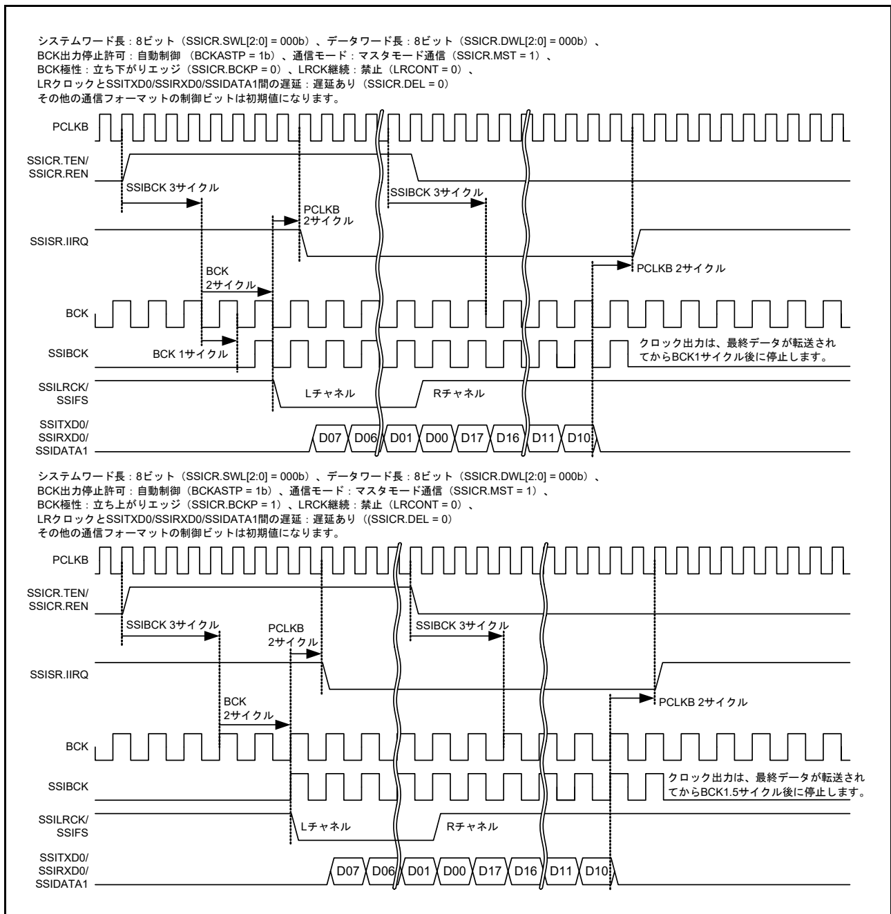
図 41.35 BCKASTP ビットの動作例 (BCKASTP = 1 での通信動作の場合)
