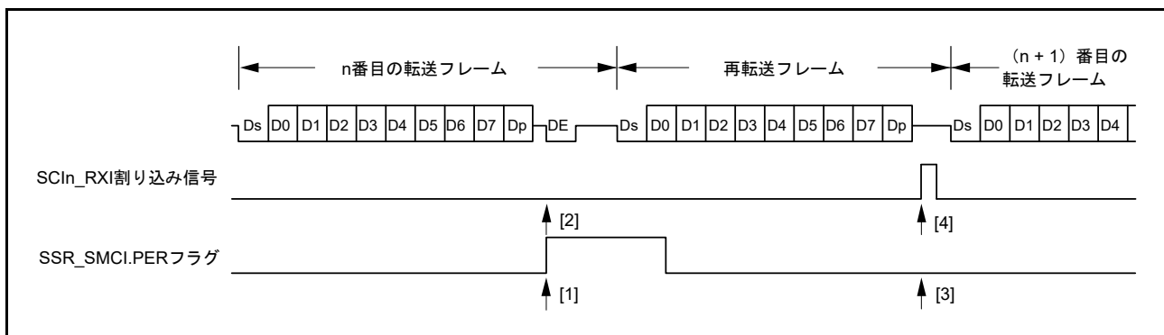
図 34.55 SCI 受信モードでの再転送動作
