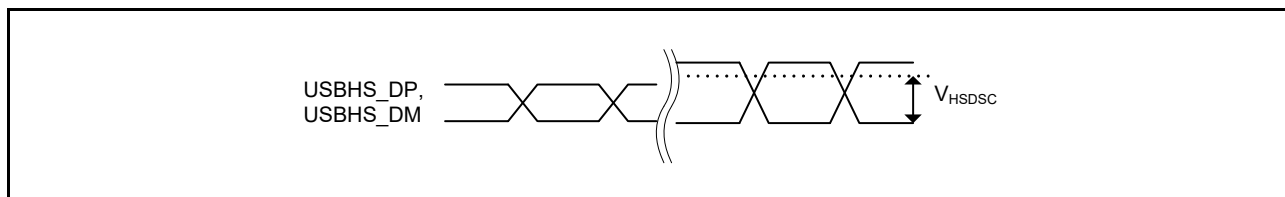
図 60.88 ハイスピードモードにおける USBHS_DP、USBHS_DM の切断検出感度
