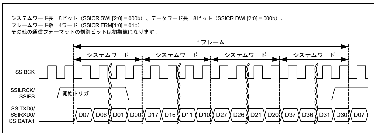
図 41.41 TDM フォーマット (パディングなし、システムワード長 = データワード長)
