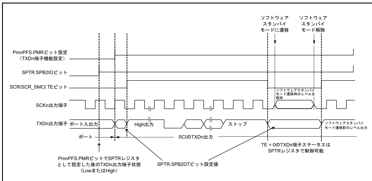
図 34.74 ソフトウェアスタンバイモード遷移中のポートの端子状態 (内部クロック、調歩同期送信)
