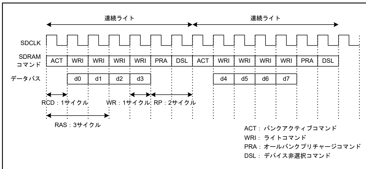
図 15.67 連続ライトタイミング例 (1)
