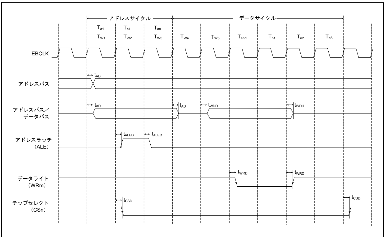
図 60.21 アドレス/データマルチプレクスバスのライトアクセスタイミング
