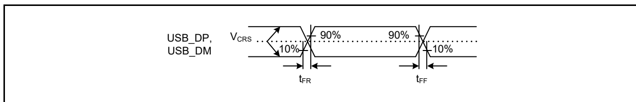
図 60.93 フルスピードモードにおける USB_DP、USB_DM の出力タイミング
