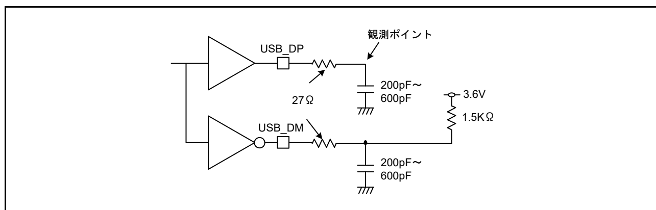
図 60.92 ロースピードモードにおける測定回路
