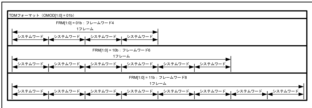
図 41.13 フレームワード数
