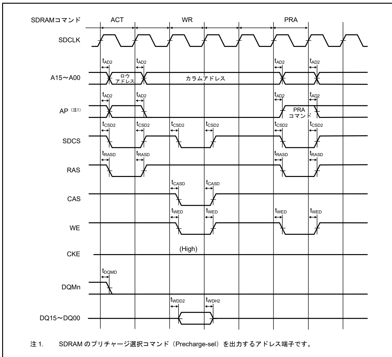
図 60.28 SDRAM シングルライトタイミング
