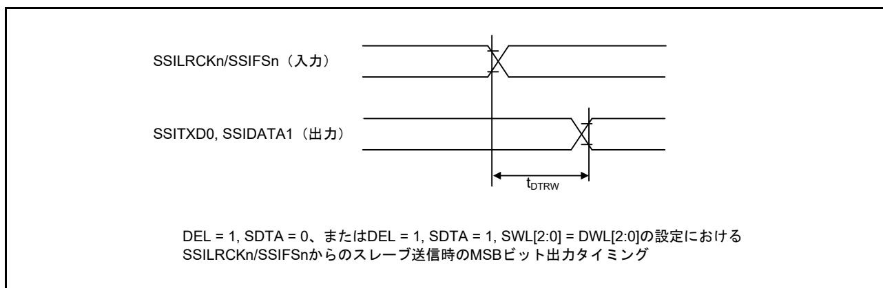
図 60.65 SSILRCKn/SSIFSn 変化時からの SSIE データ出力遅延
