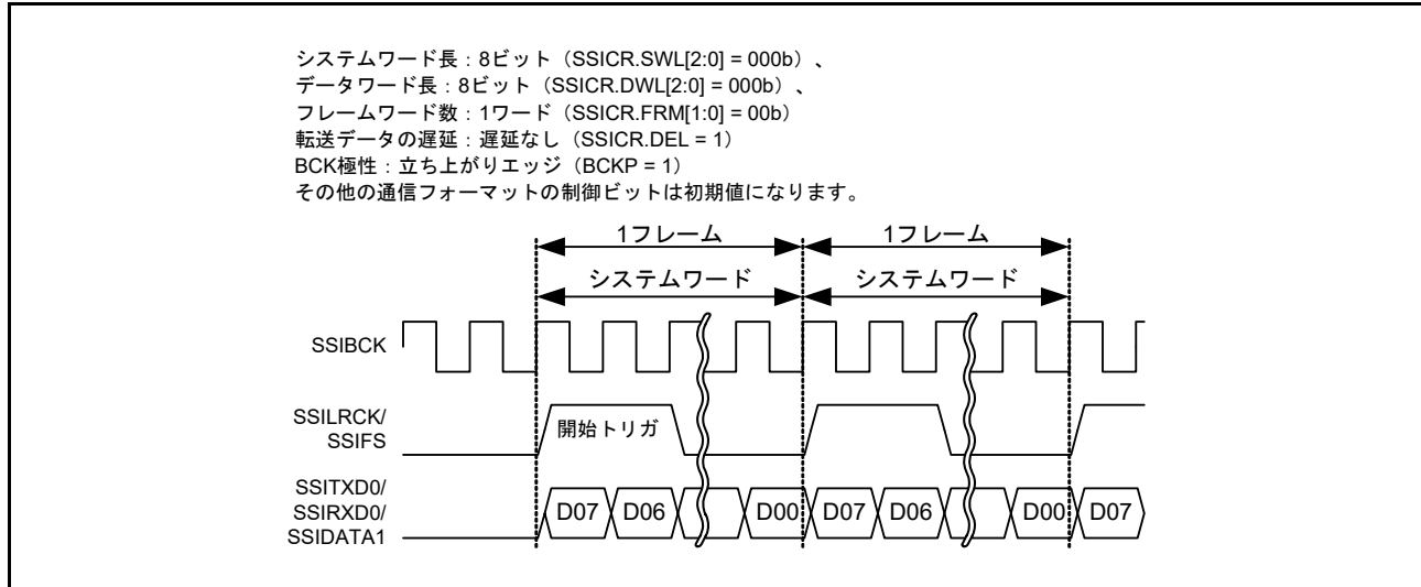
図 41.40 モノラルフォーマットでのロングフレーム (パディングなし)
