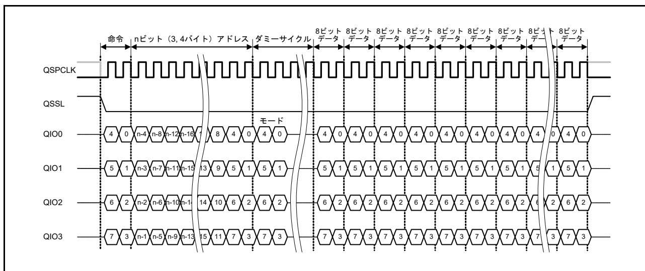
図 39.7 Quad-SPI プロトコル例 (ファストリード Quad I/O)
