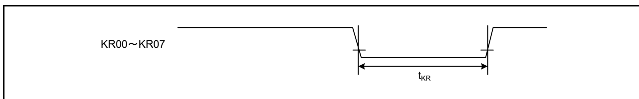
図 60.42 キー割り込み入力タイミング
