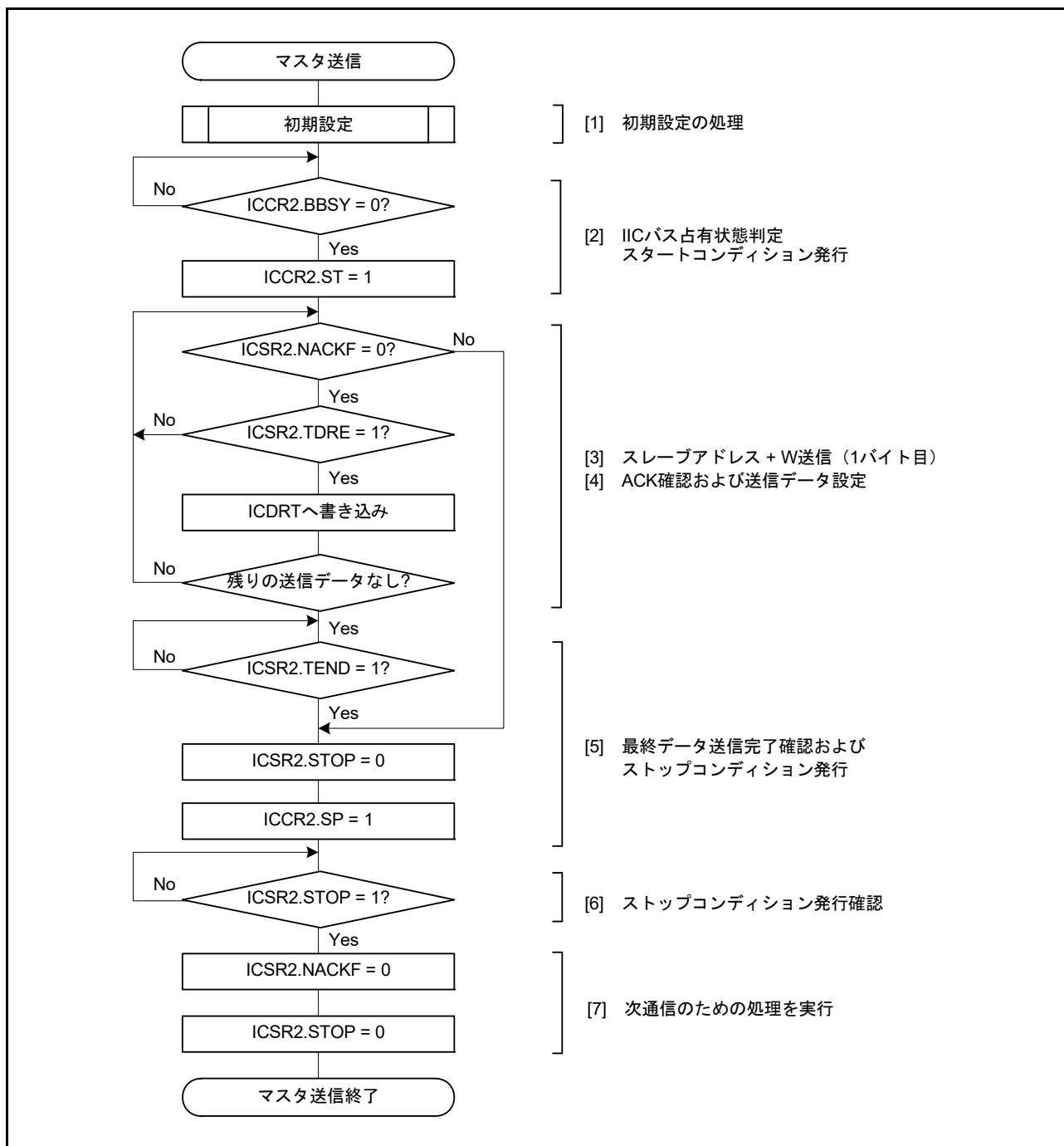
図 36.6 マスタ送信のフロー例
