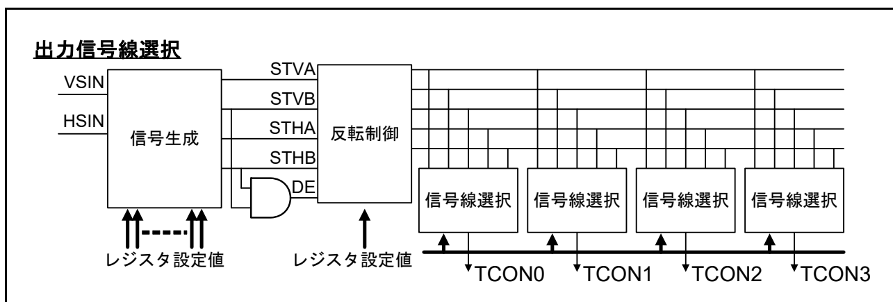
図 58.19 反転制御と出力信号選択の構成
