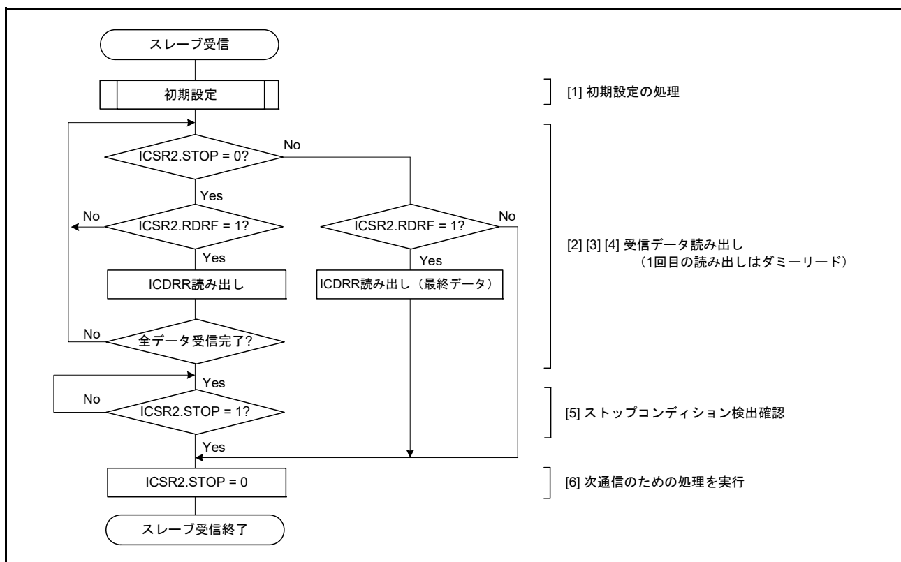
図 36.18 スレーブ受信のフロー例
