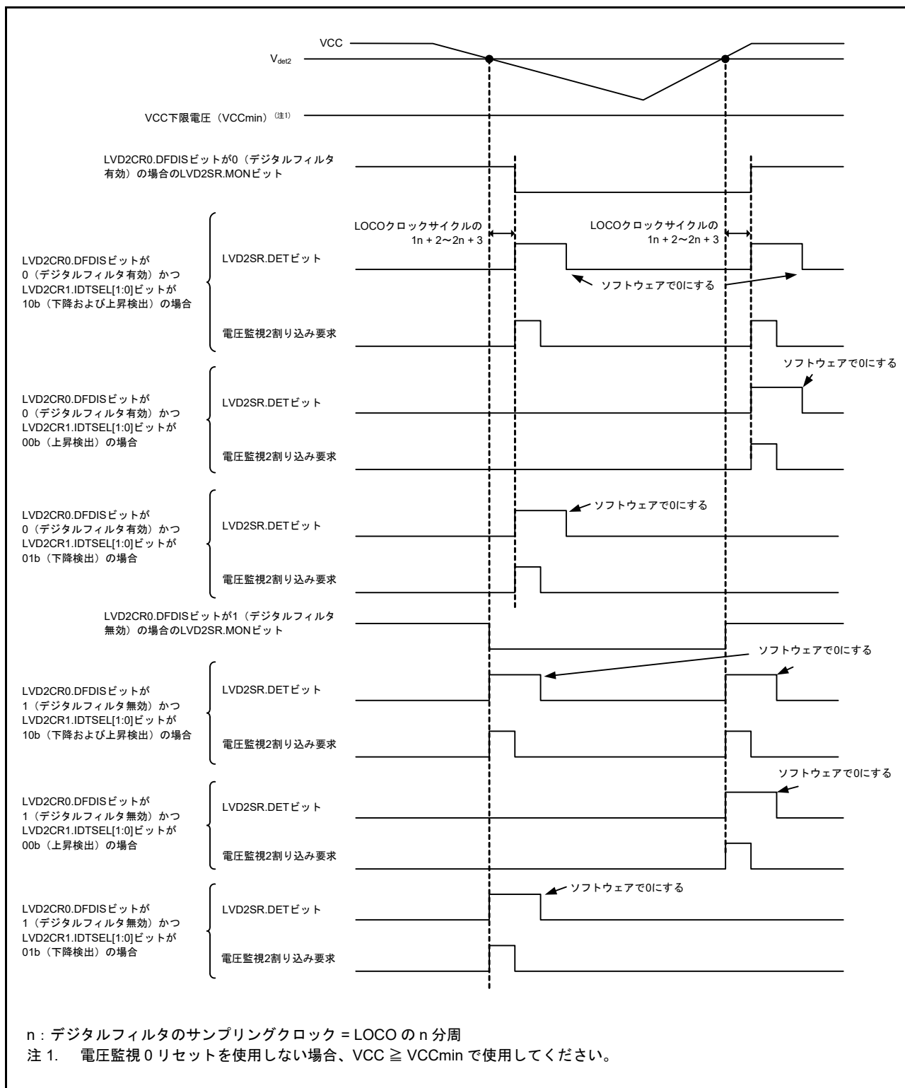
図 8.6 電圧監視 2 割り込みの動作例
