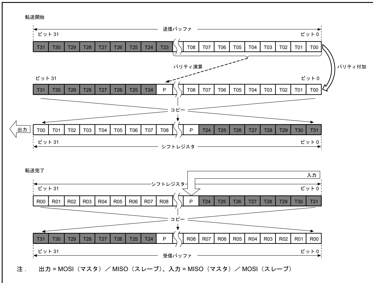
図 38.21 LSB ファースト転送 (24 ビットデータ/パリティ機能有効)
