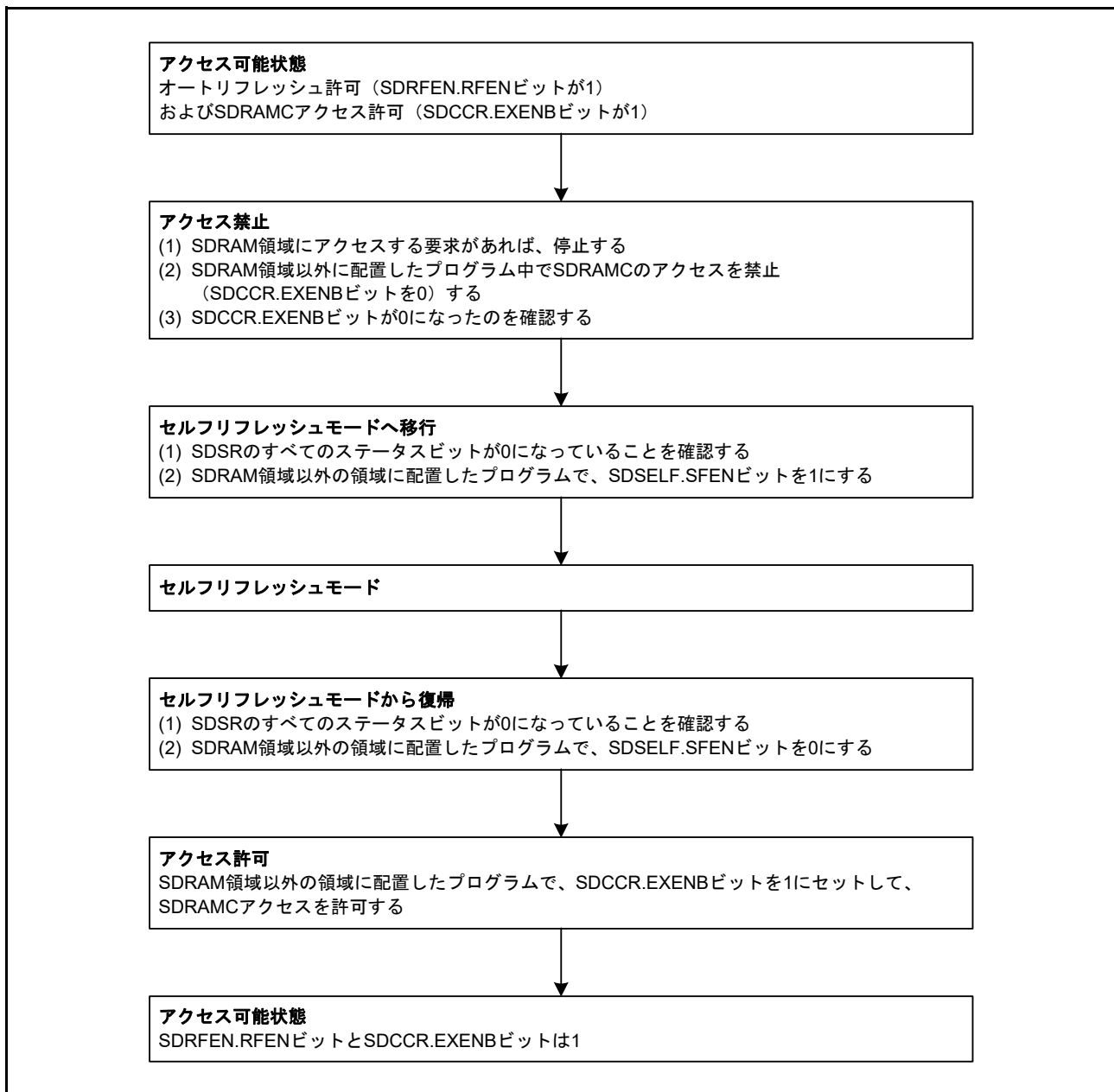
図 15.52 セルフリフレッシュモード遷移／復帰手順
