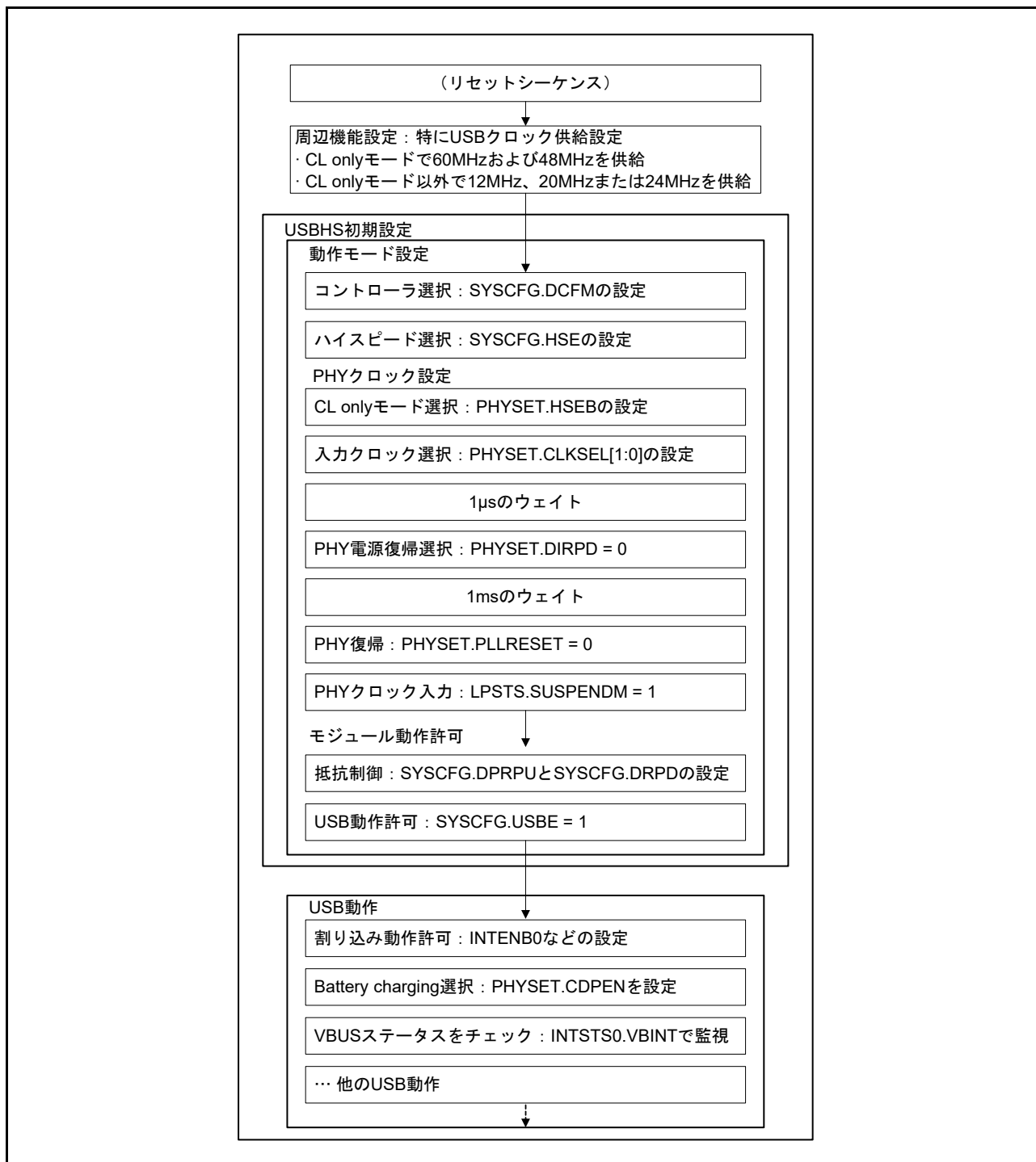
図 33.2 PHY クロック設定
