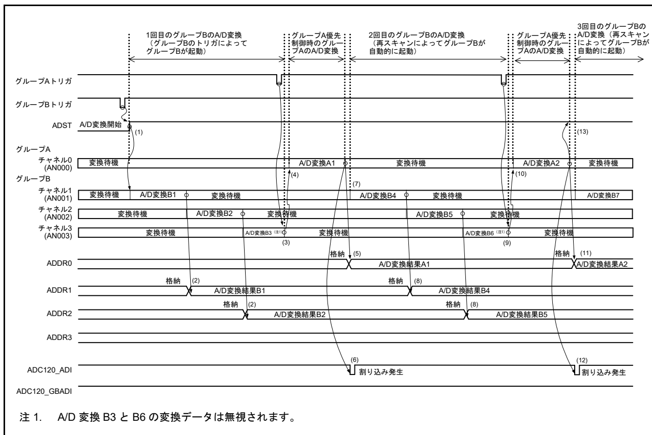
図 47.27 グループ A 優先制御の動作例 (2) (ADGSPCR.GBRSCN = 1、ADGSPCR.GBRP = 0 の場合)
