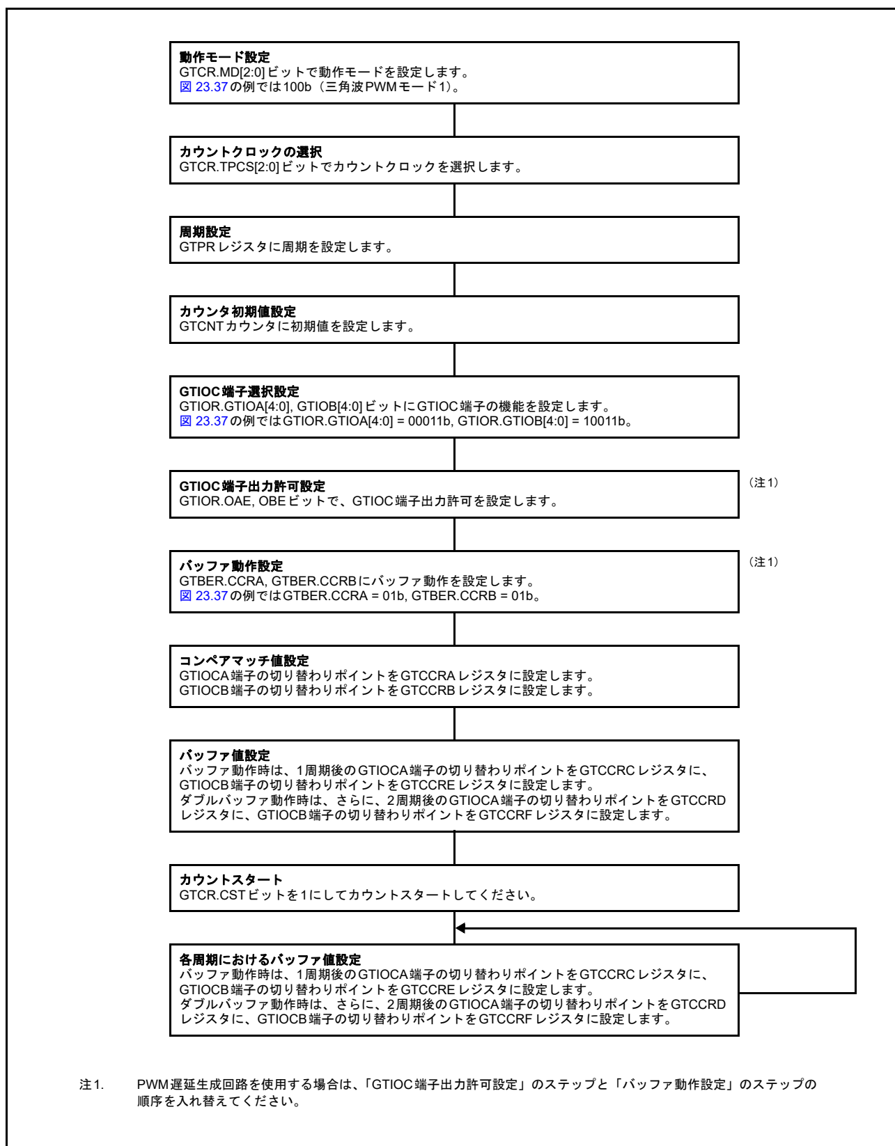
図 23.38 三角波 PWM モード 1 設定例
