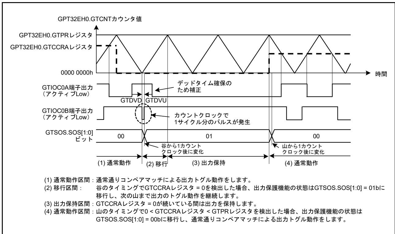
図 23.101 山でのバッファ転送中に GTCCR レジスタが 0 になった場合の出力保護機能の動作例 (山でのバッファ転送中に 0 < \text{GTCCR レジスタ} < \text{GTPR レジスタ} を回復、アクティブ Low の場合)
