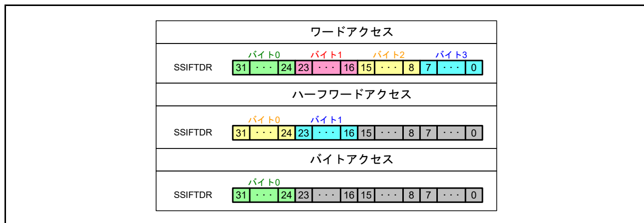
図 41.30 送信 FIFO データレジスタへのレジスタアクセス例
