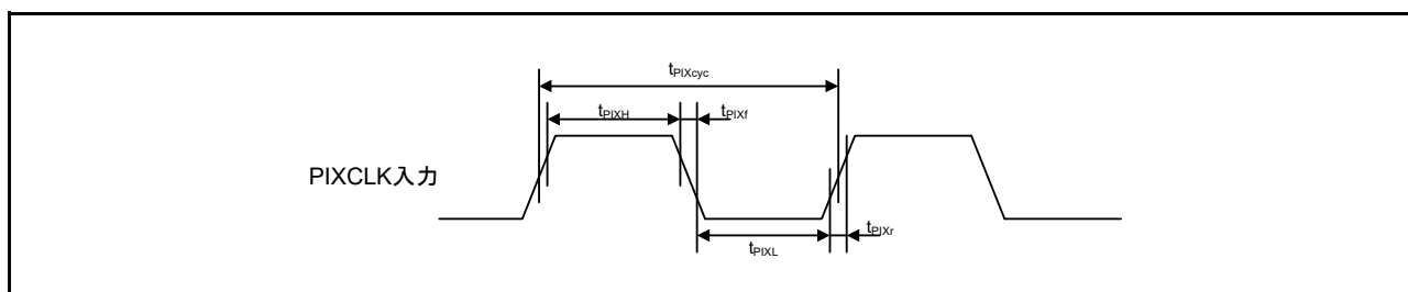
図 60.77 PDC 入力クロックタイミング
