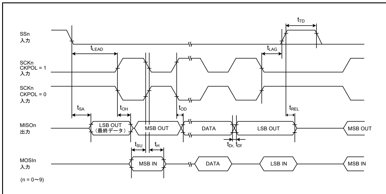
図 60.49 CKPH = 0 の場合におけるスレーブの SCI 簡易 SPI モードタイミング
