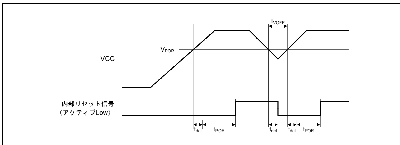
図 60.97 パワーオンリセットタイミング
