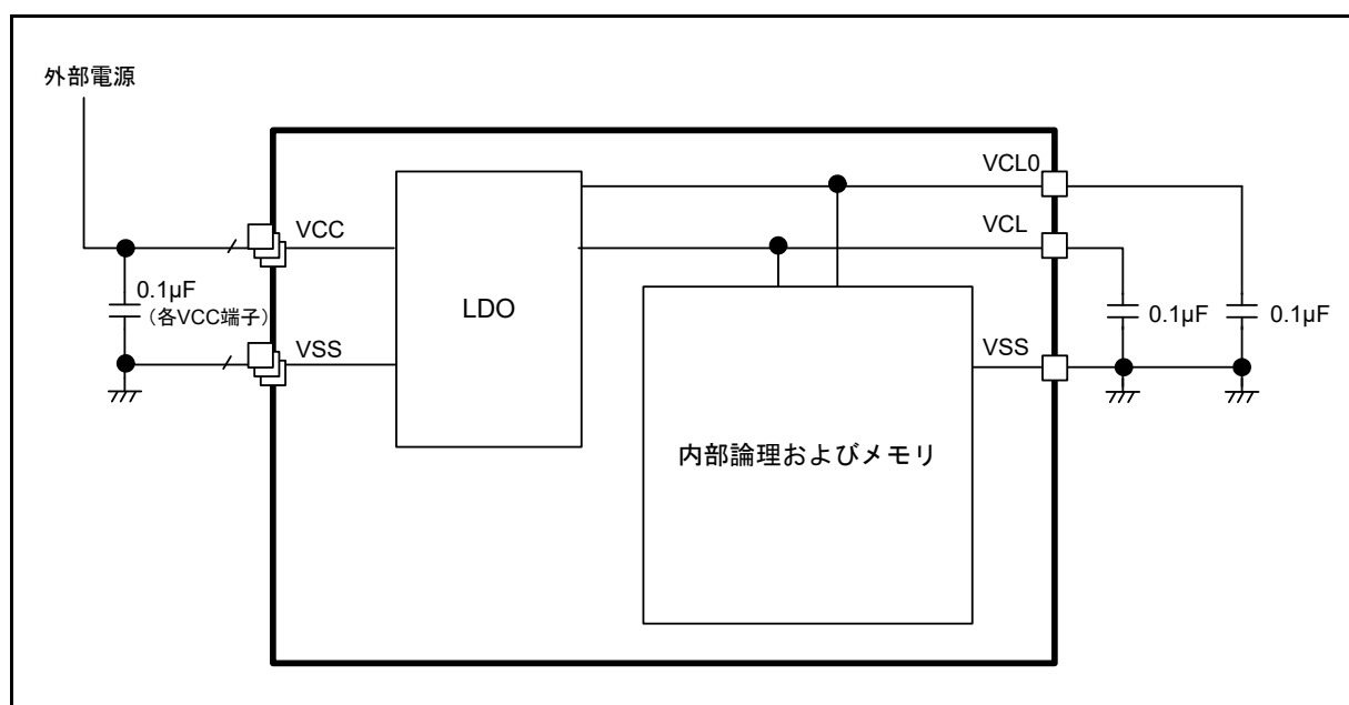
図 59.1 LDOモード設定
