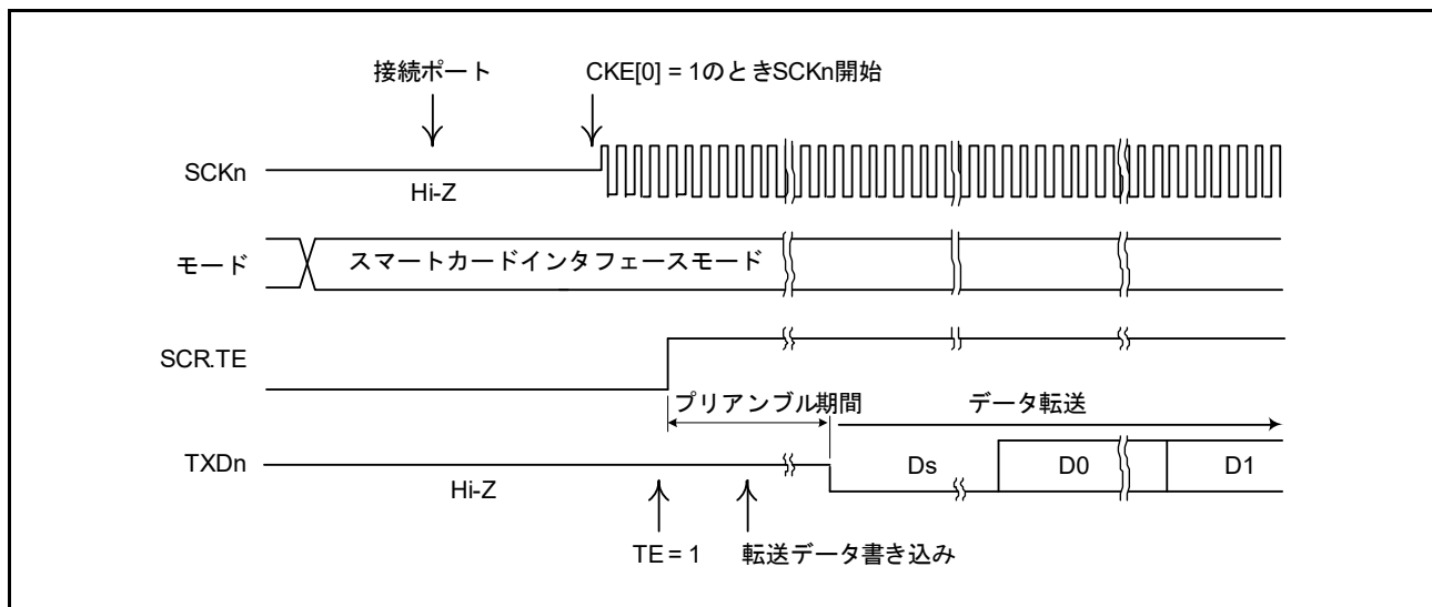
図 34.51 スマートカードインタフェースモードにおけるデータ送信のタイミング例
