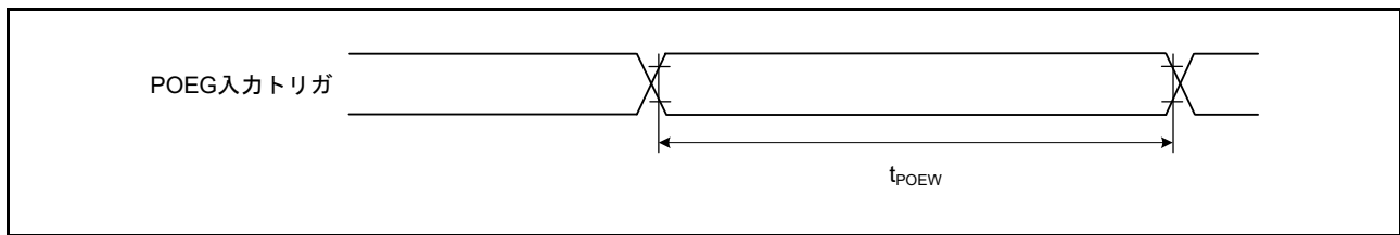
図 60.35 POEG 入力トリガタイミング
