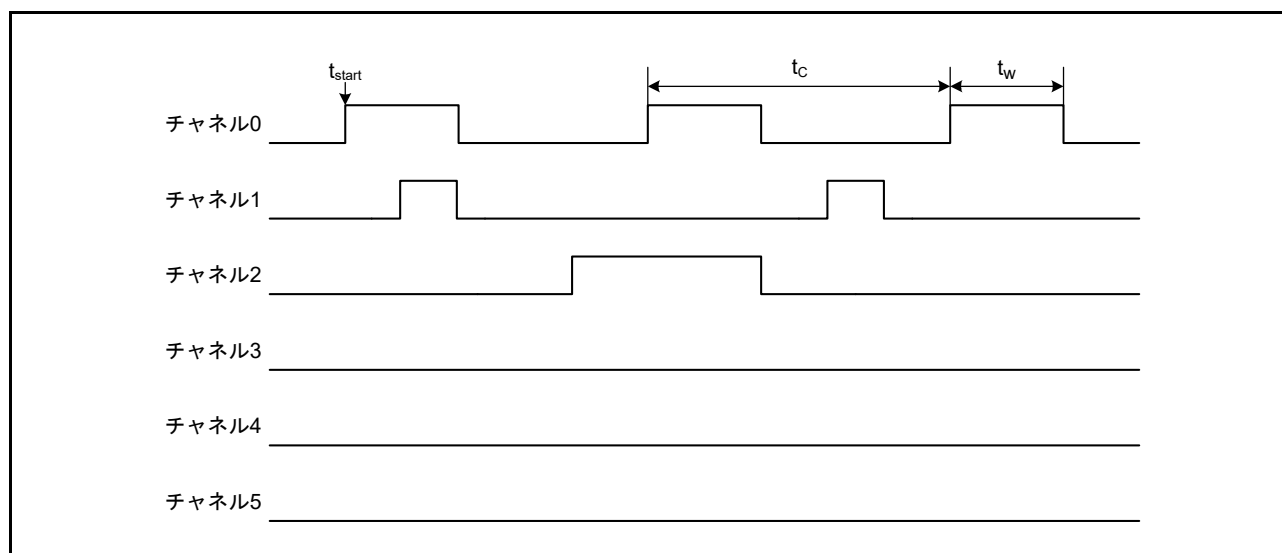
図 30.28 パルス出力タイマの動作タイミング
