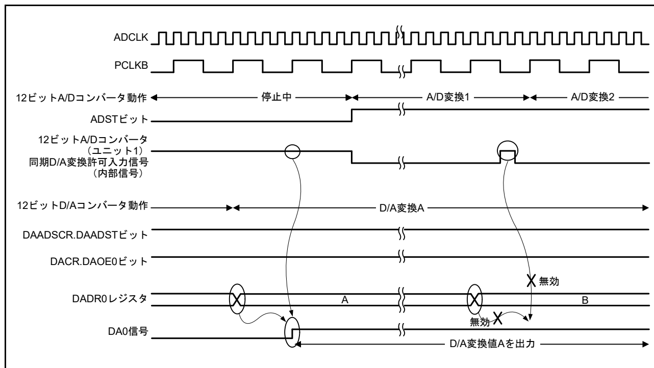
図 48.4 DAC12 が ADC12 (ユニット 1) からの同期 D/A 変換許可入力信号を取り込めない場合の例
