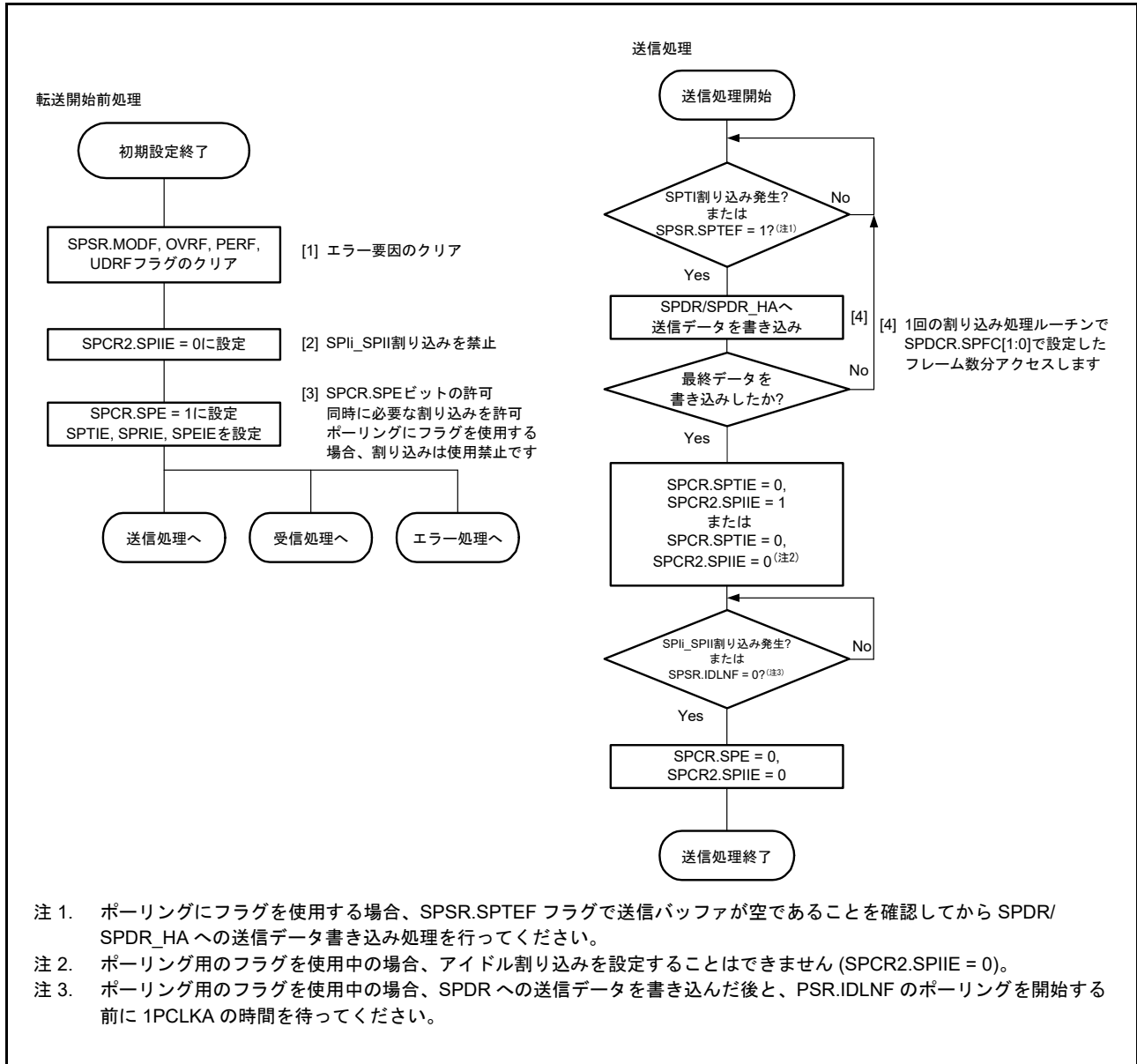
図 38.37 マスタモードでの送信フロー
