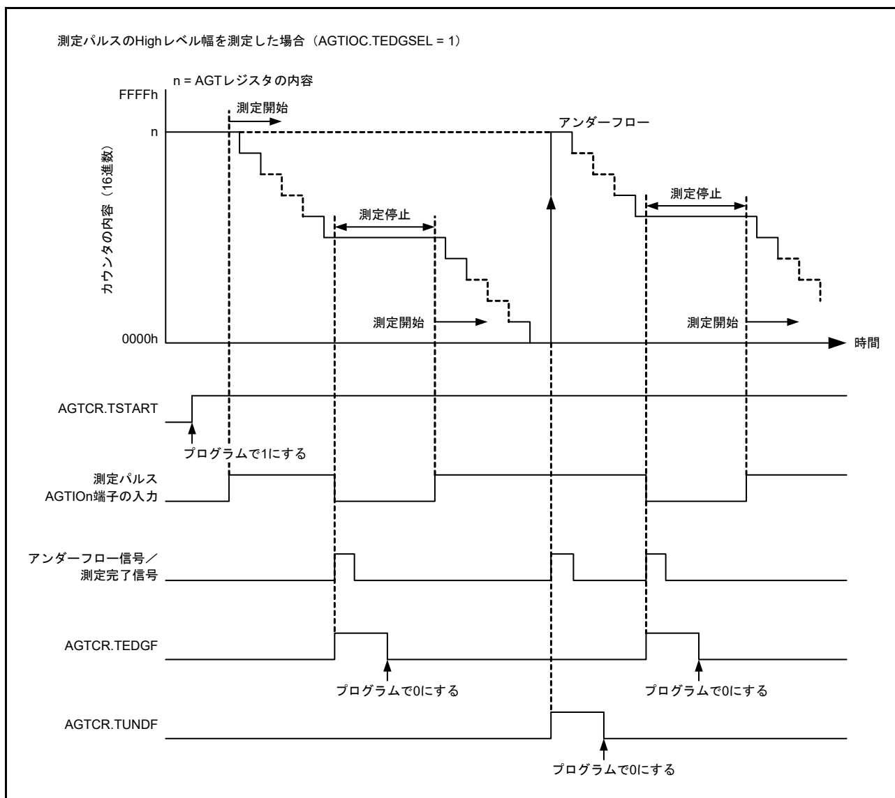
図 25.9 パルス幅測定モードでの動作例
