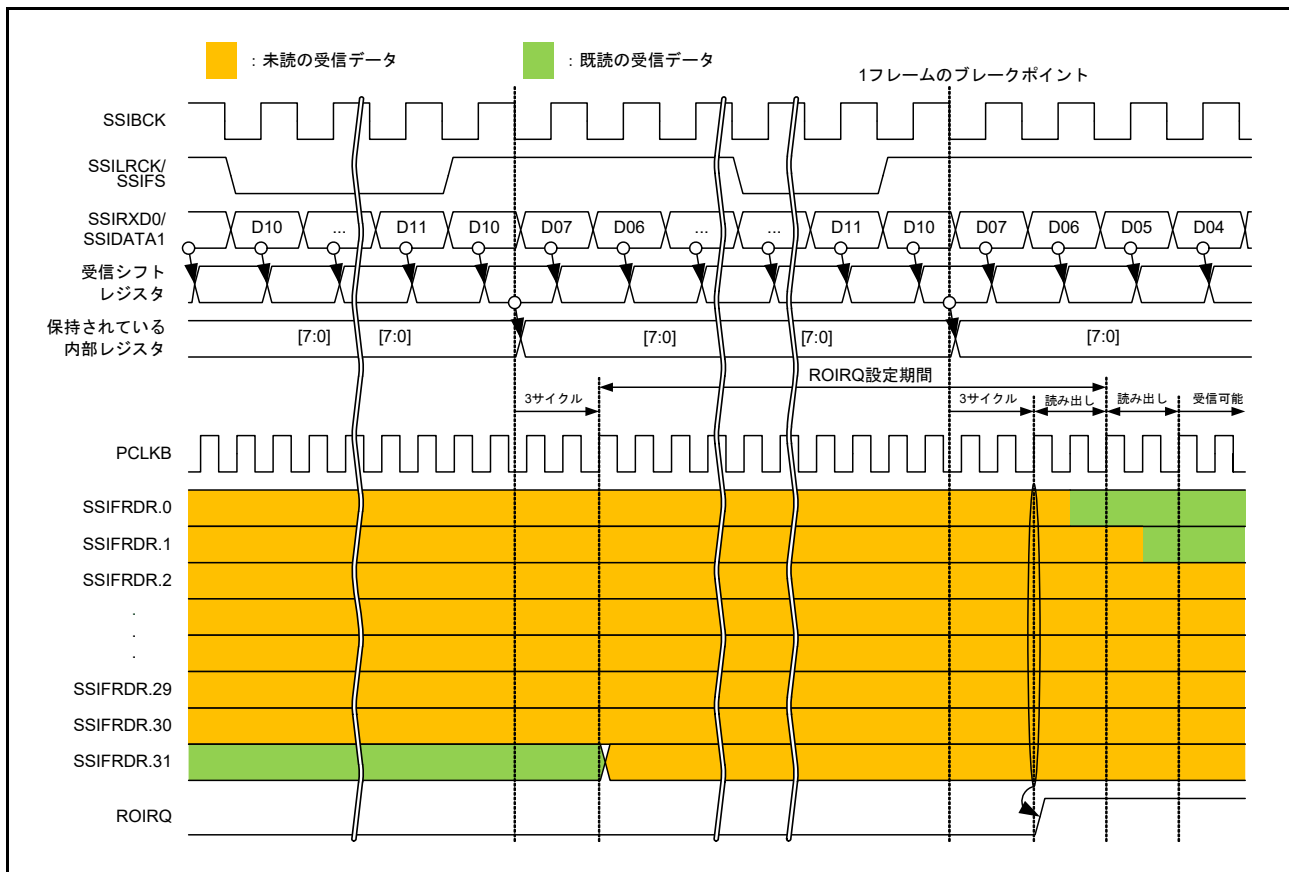
図 41.16 ROIRQ 設定タイミング
