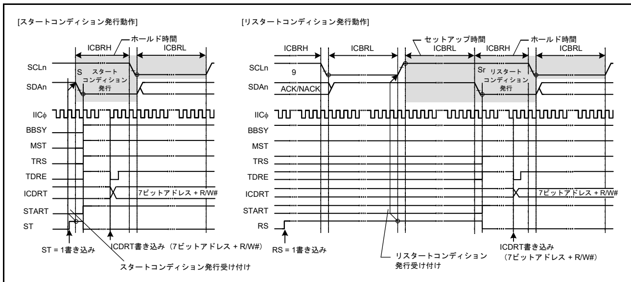
図 36.45 スタートコンディション、リスタートコンディションの発行動作タイミング (ST および RS ビットの使用)
