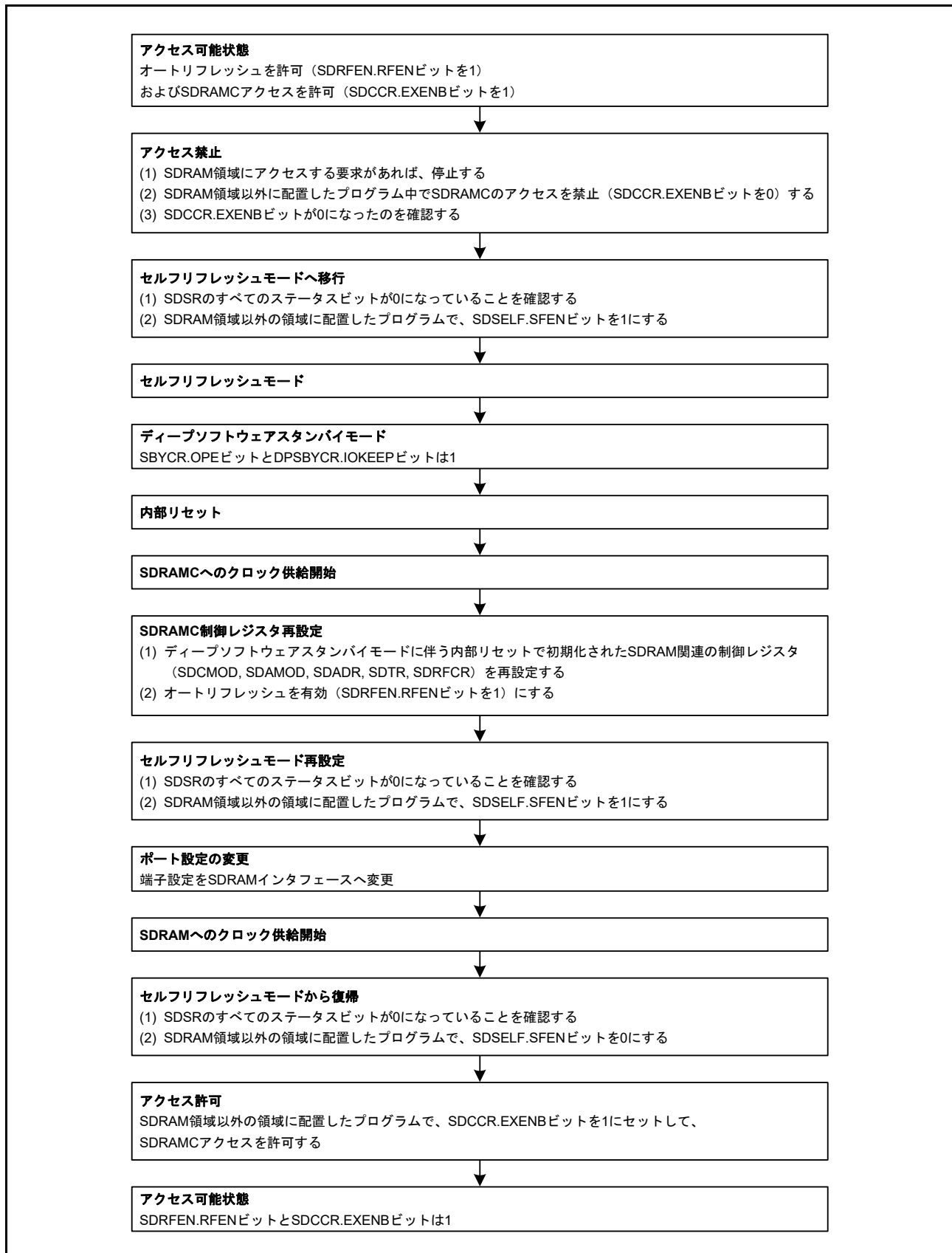
図 15.53 ディープソフトウェアスタンバイモードでのセルフリフレッシュモード遷移/復帰手順
