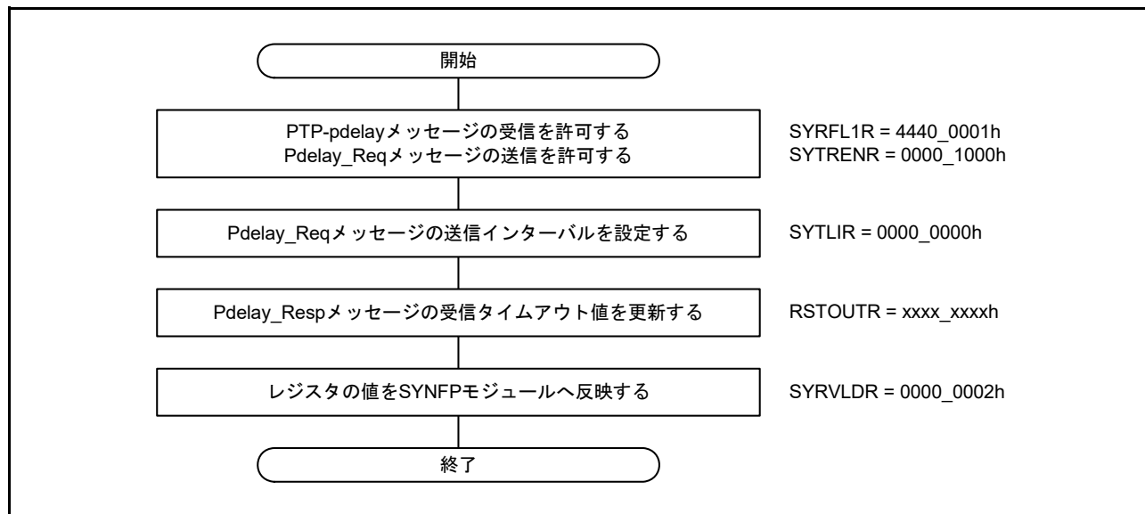
図 30.14 P2P 動作開始手順
