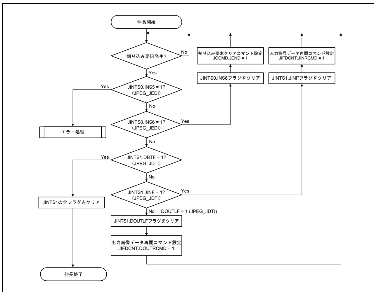
図 57.9 伸長処理フロー
