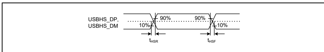
図 60.89 ハイスピードモードにおける USBHS_DP、USBHS_DM の出カタイミング
