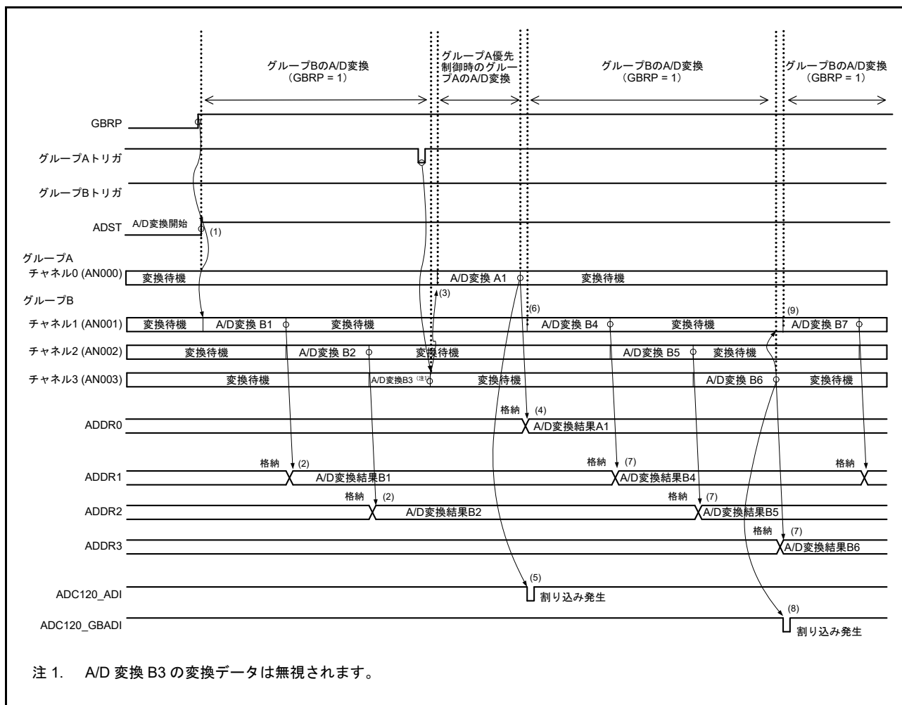
図 47.30 グループ A 優先制御の動作例 (5) (ADGSPCR.GBRP = 1 の場合)
