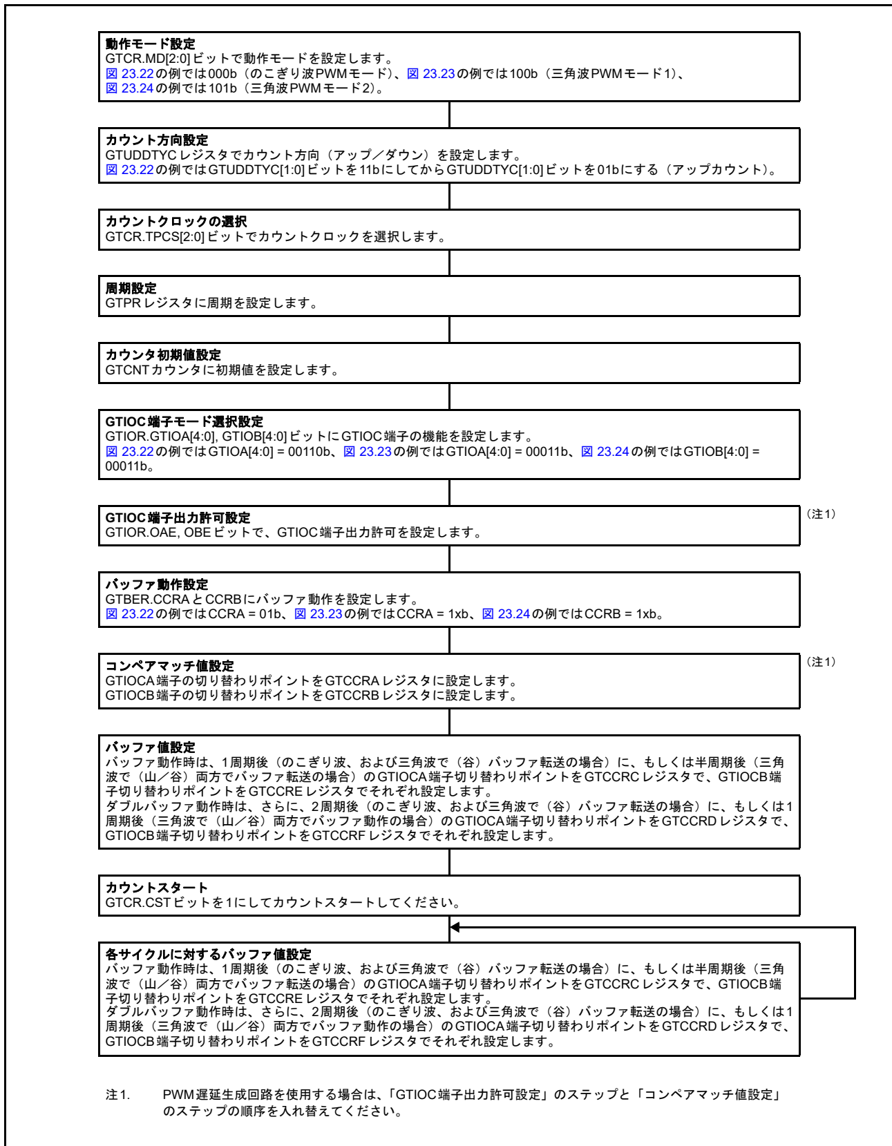
図 23.25 GTCRA、GTCCRB レジスタのバッファ動作設定例 (アウトプットコンペア時)
