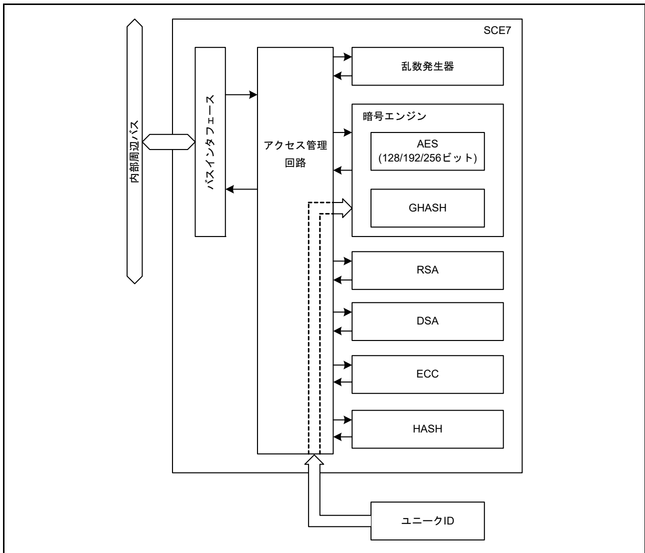
図 46.1 SCE7 ブロック図
