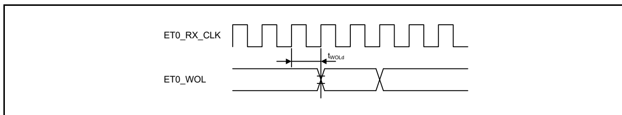
図 60.76 MII に対する WOL 出力タイミング
