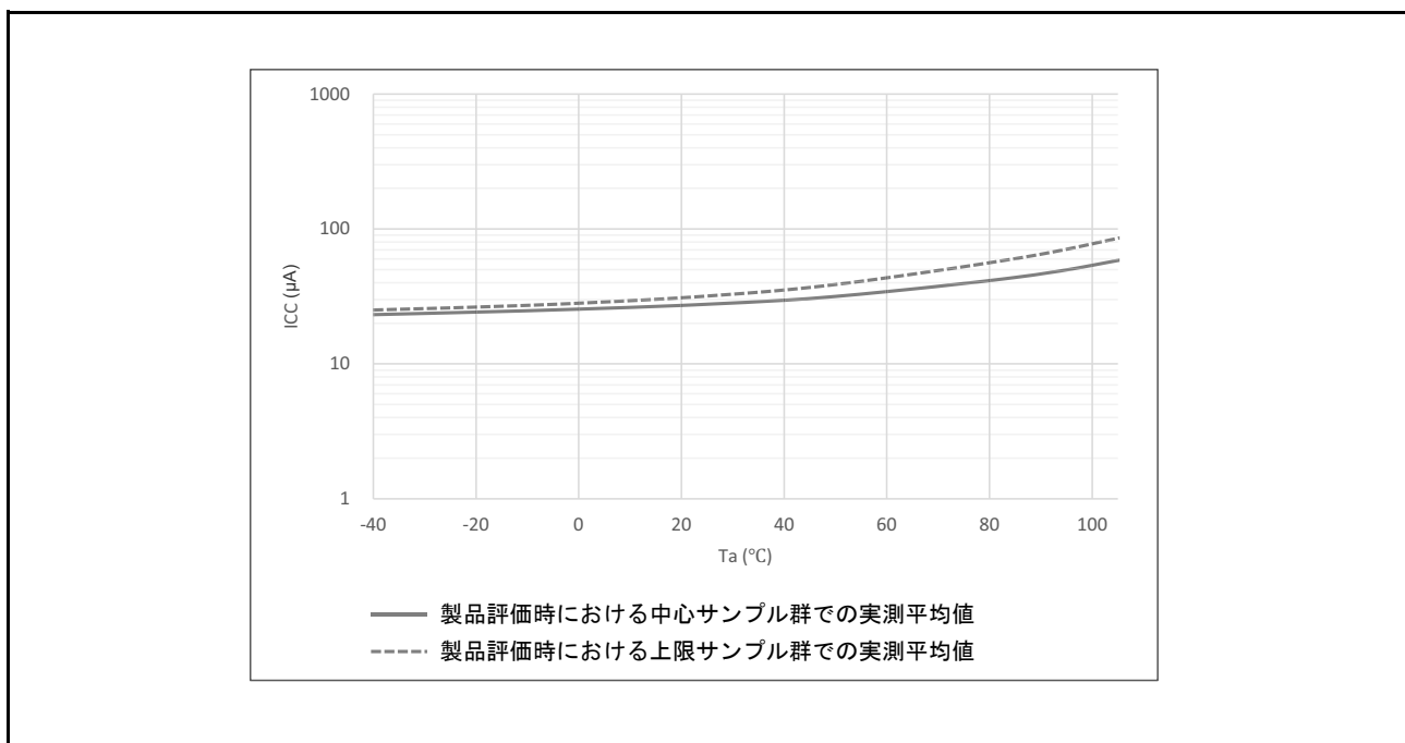
図 60.3 ディープソフトウェアスタンバイモード時にスタンバイ SRAM および USB レジューム検出部へ電源を供給する場合の温度依存性 (参考データ)
