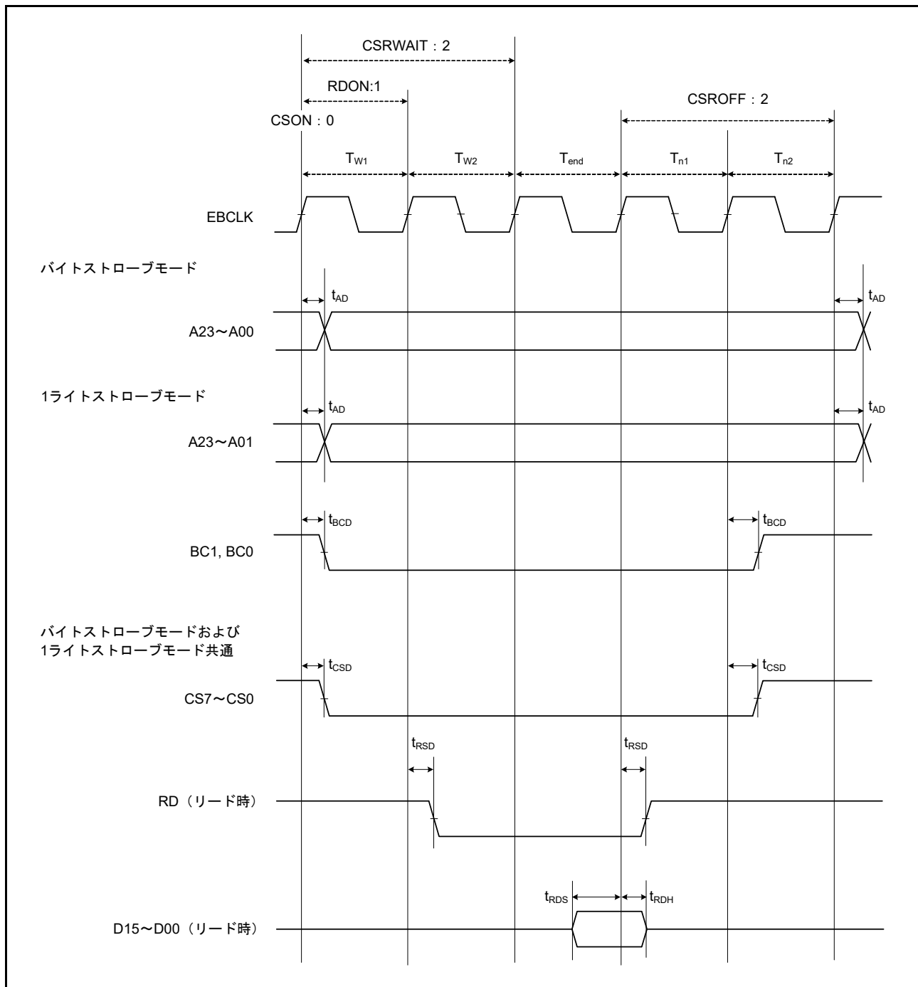
図 60.22 バスクロック同期を使用したノーマルリードサイクルの外部バスタイミング
