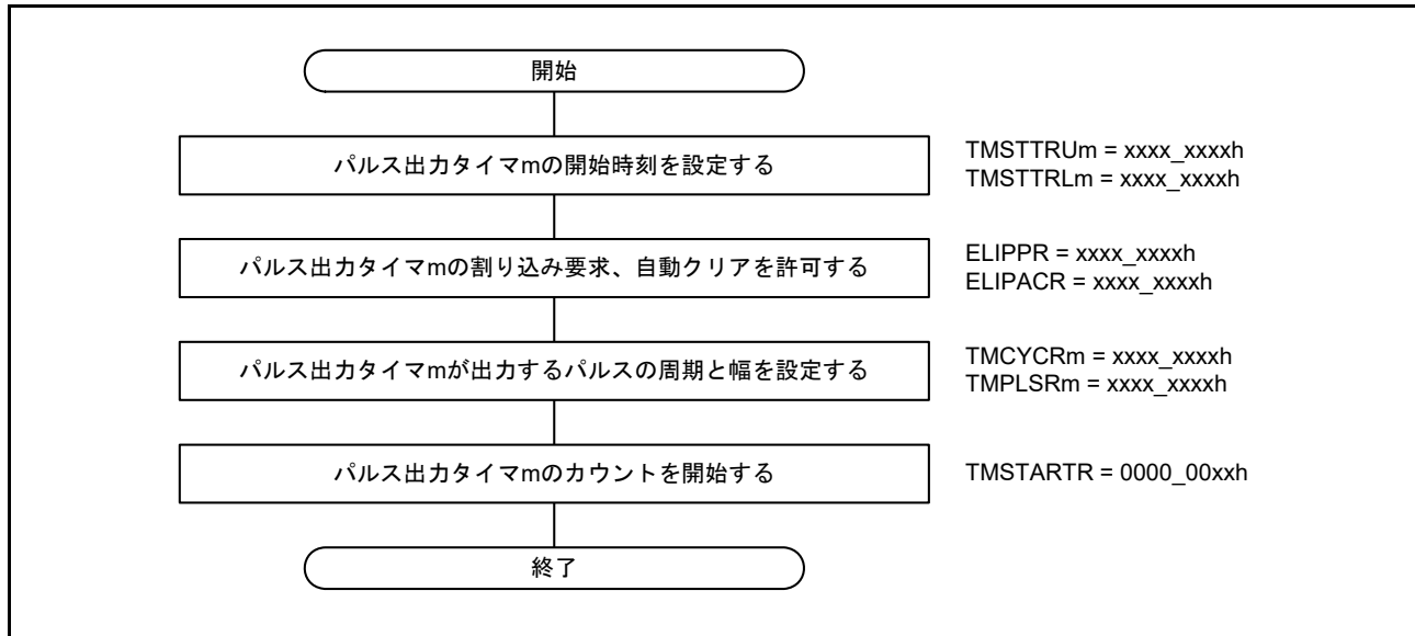
図 30.29 パルス出力タイマ設定手順
