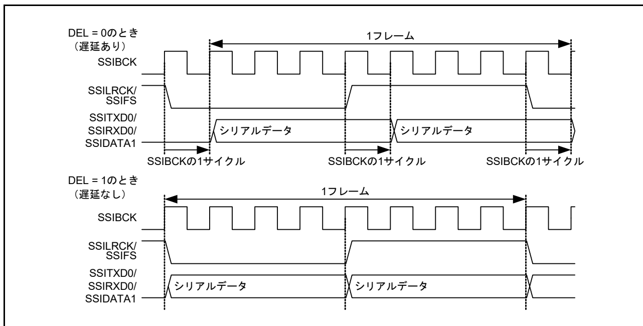
図 41.7 シリアルデータディレイの設定
