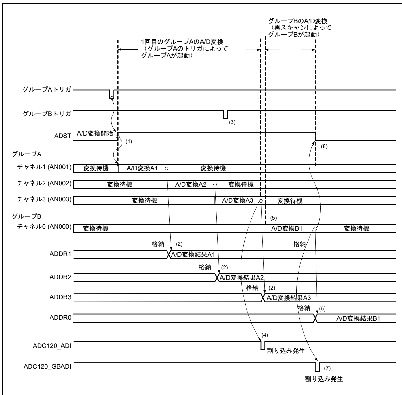
図 47.28 グループ A 優先制御の動作例 (3) (ADGSPCR.GBRSCN = 1、ADGSPCR.GBRP = 0 の場合)
