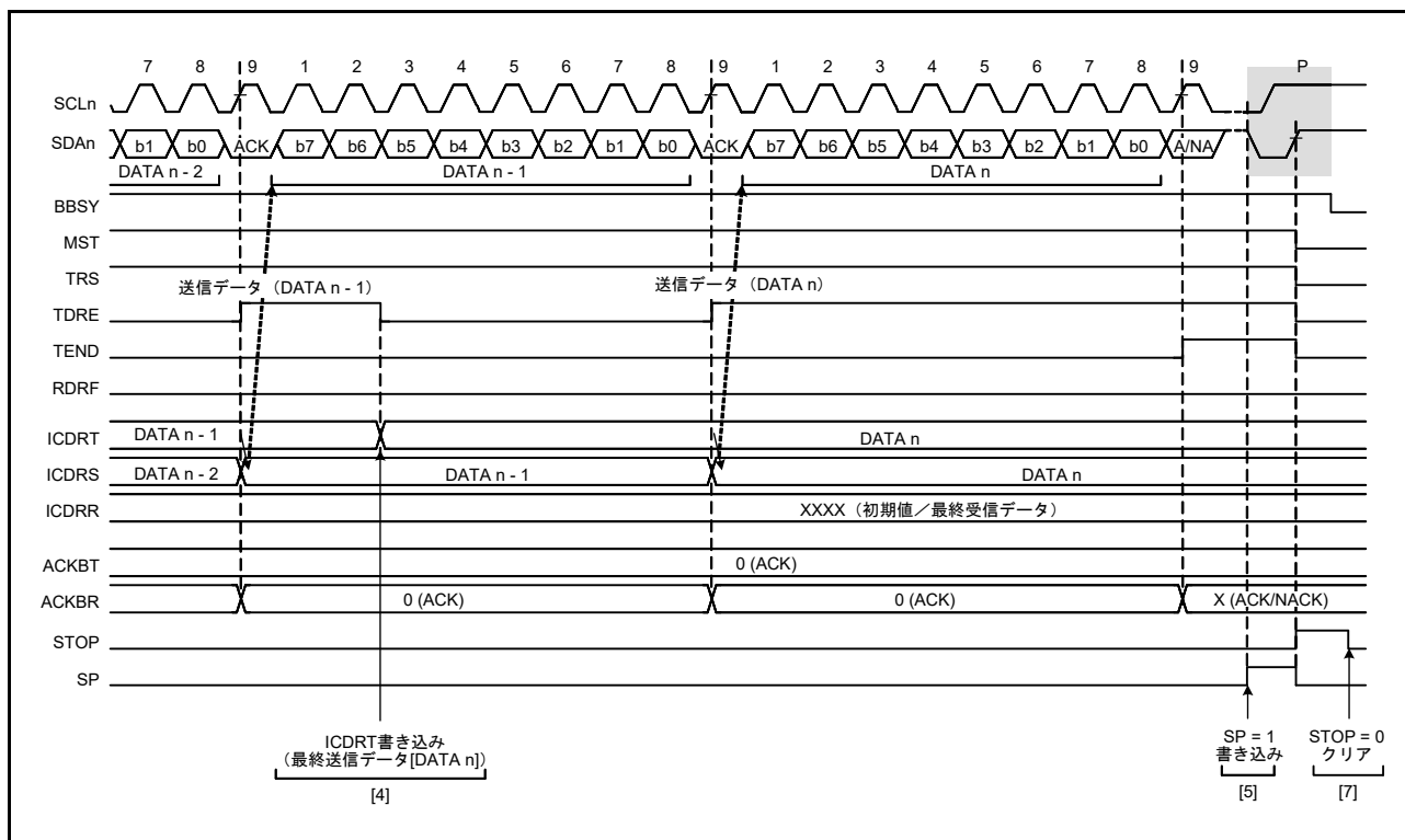
図 36.9 マスタ送信の動作タイミング (3)
