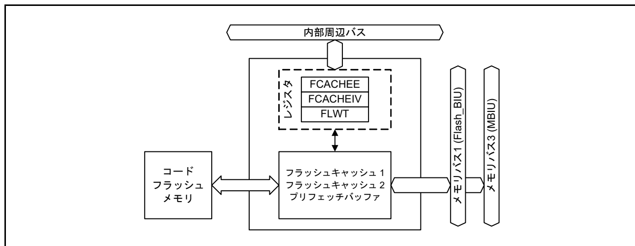
図 55.4 FCACHE のブロック図
