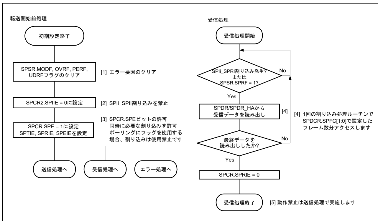
図 38.38 マスタモードでの受信フロー
