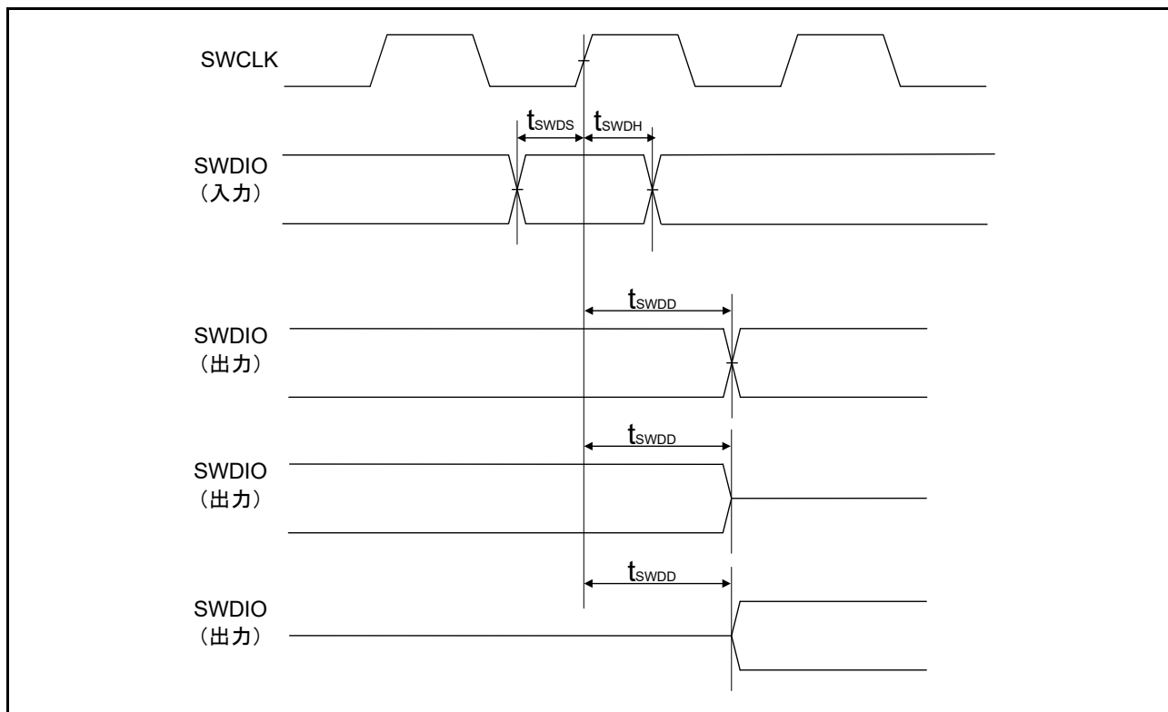
図 60.109 SWD 入出力タイミング
