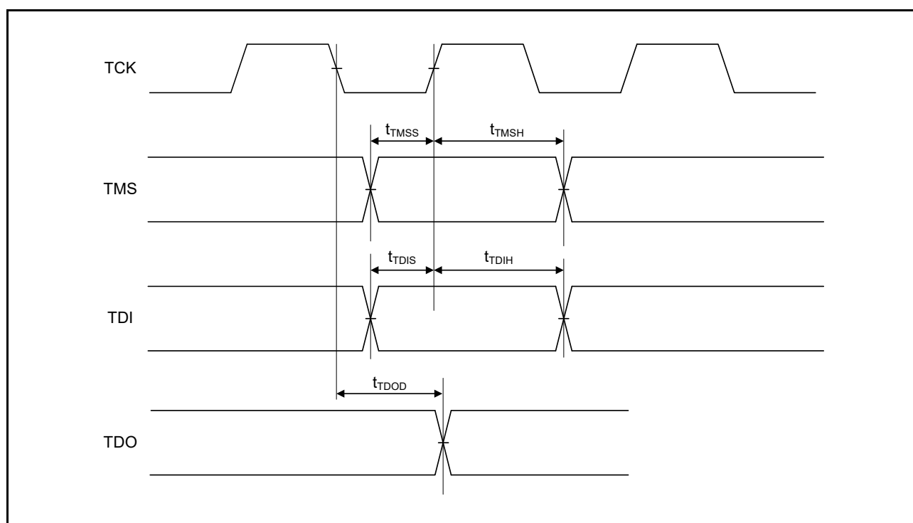
図 60.107 JTAG 入出力タイミング
