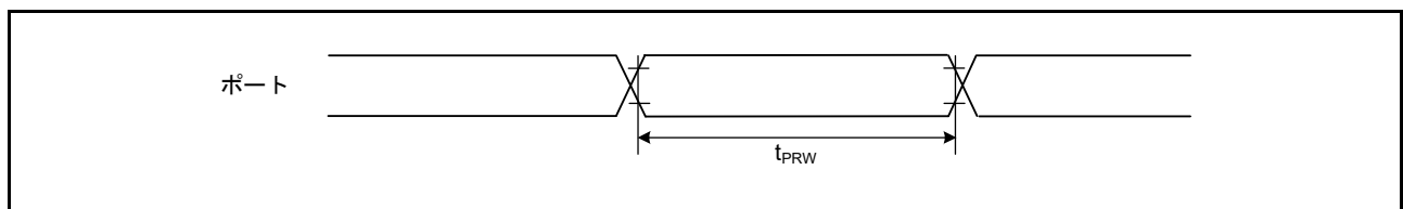
図 60.34 I/Oポート入力タイミング
