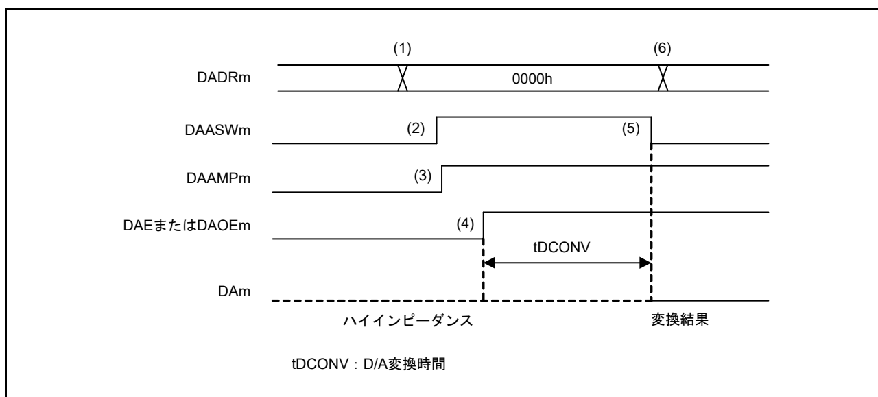
図 48.5 出力アンプを使用した DAC12 の初期化フロー例
