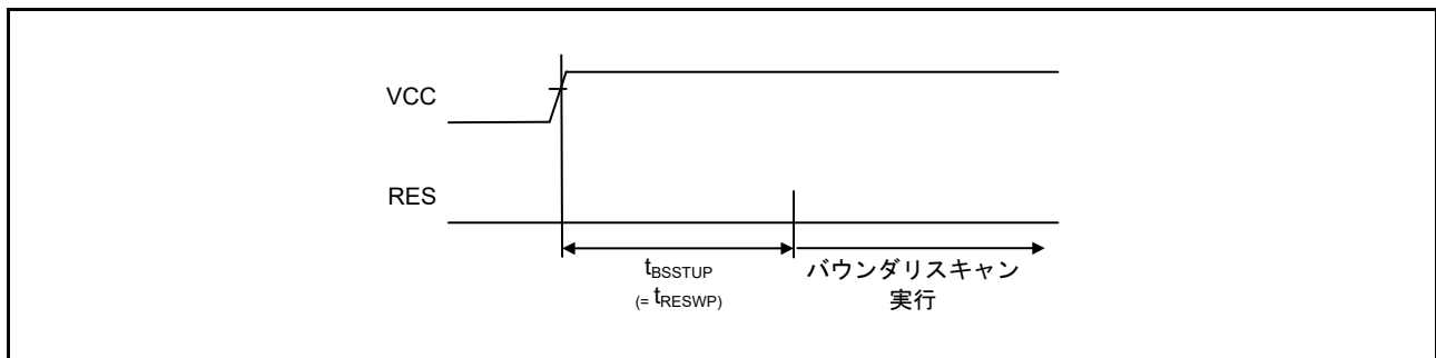
図 60.105 バウンダリスキャン回路起動タイミング
