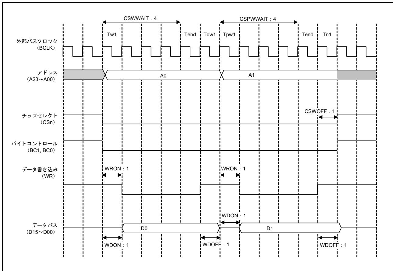
図 15.24 ページライトアクセスの動作例 (16 ビットバス空間に対する 32 ビットアクセスの場合、1 ライトストロブモード時) (n = 0 ~ 7)
