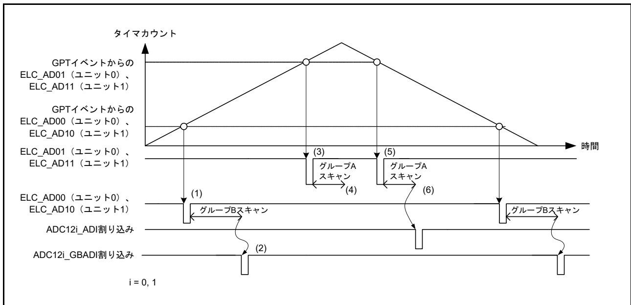
図 47.24 グループスキャンモードでダブルトリガモードを使用する場合の基本動作例 (ELC からの同期トリガ使用時)
