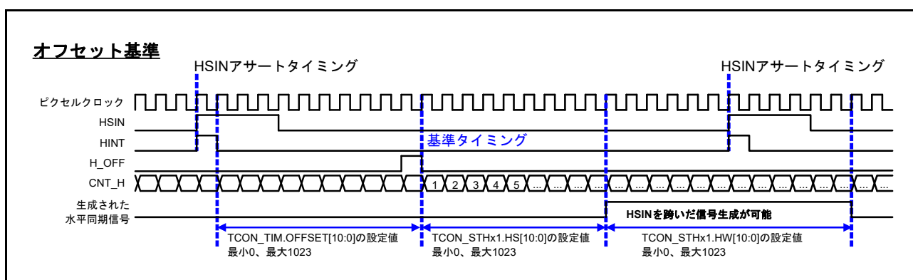
図 58.21 オフセットに基づく水平同期信号の生成
