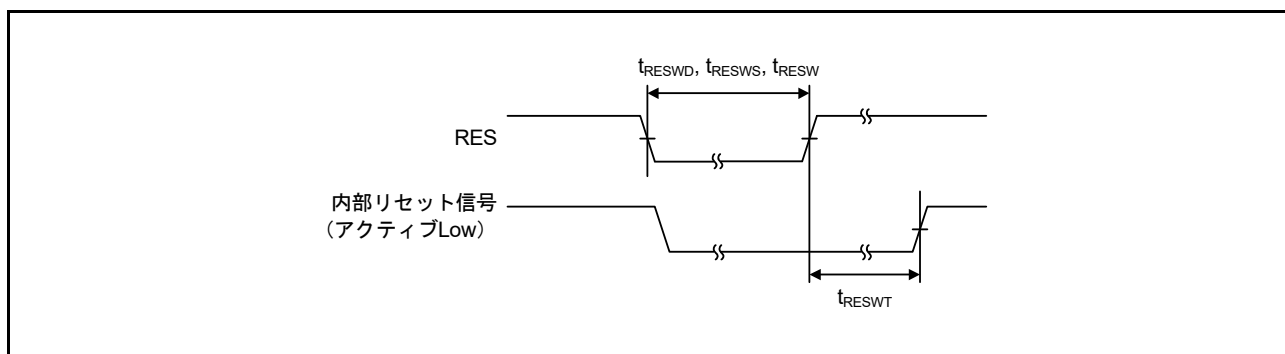
図 60.14 リセット入力タイミング
