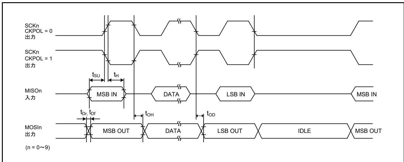
図 60.46 CKPH = 1 の場合におけるマスタの SCI 簡易 SPI モードタイミング
