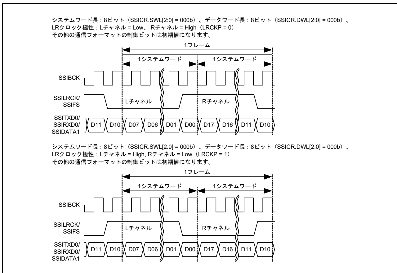
図 41.12 LRクロック/フレーム同期極性設定
