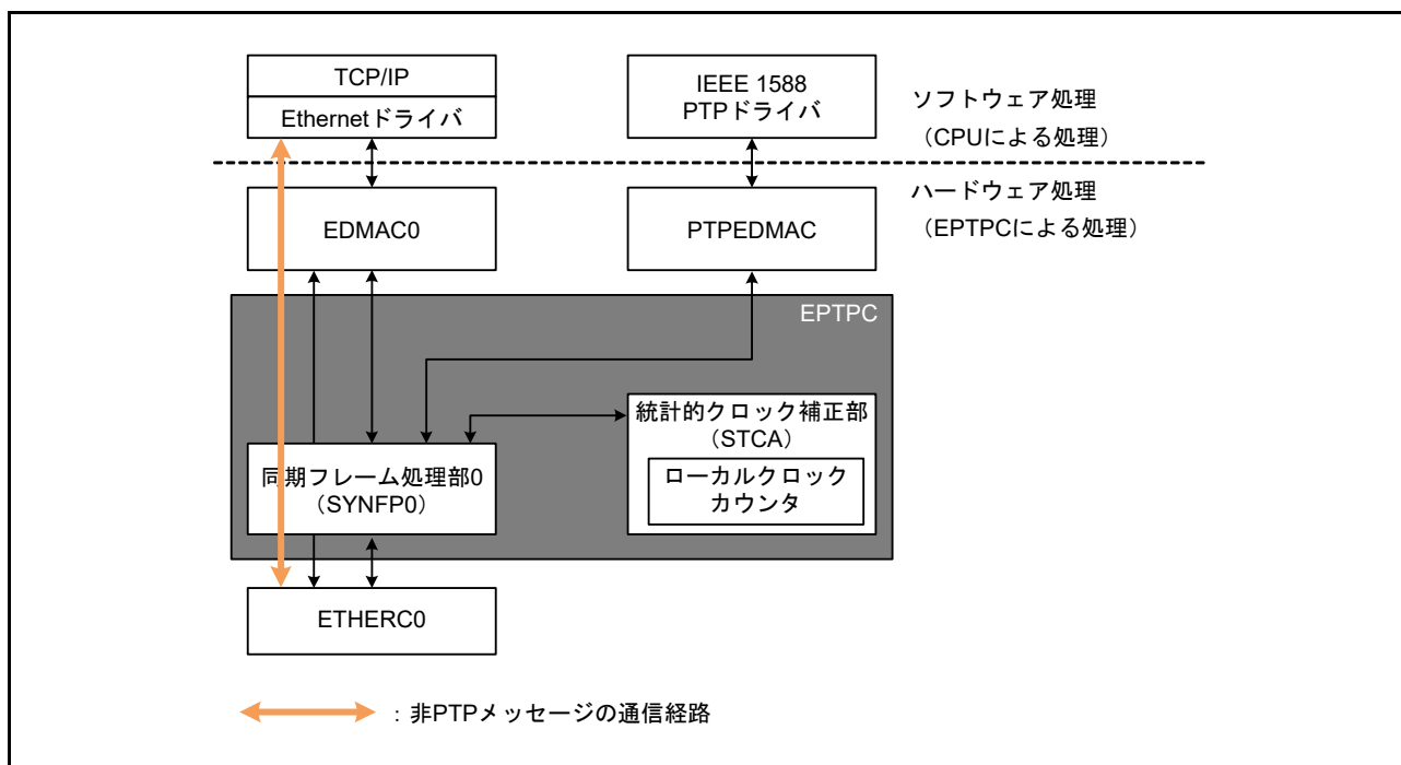
図 30.4 非 PTP メッセージの送受信の経路
