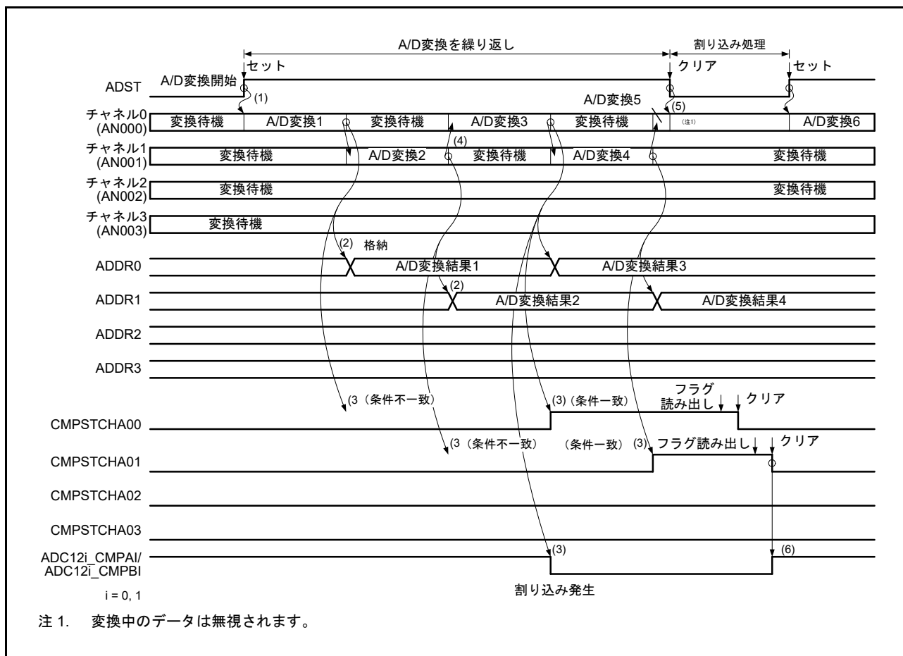
図 47.31 コンペア機能の動作例 (AN000 ~ AN003 を比較)
