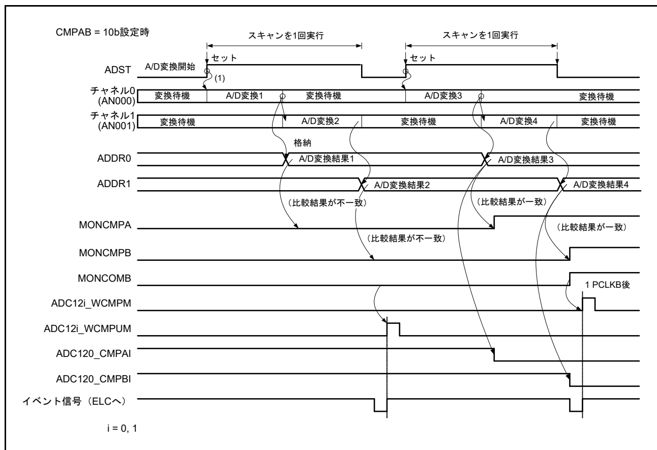
図 47.33 コンペア機能のイベント出力動作例 (AN000 ~ AN001 を比較)
