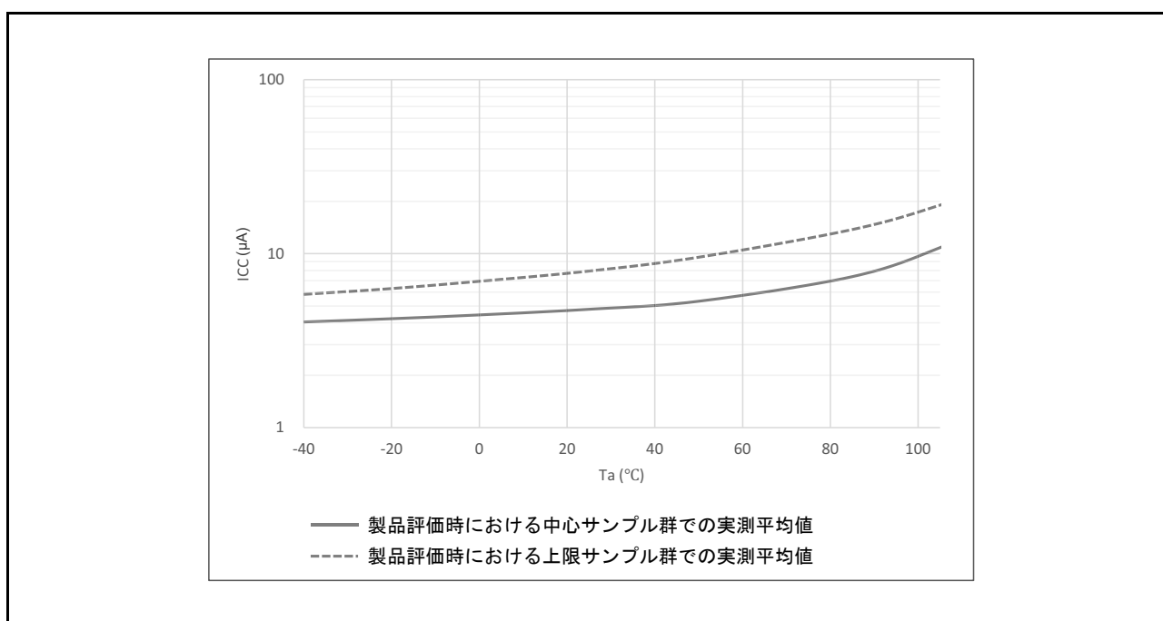
図 60.5 ディープソフトウェアスタンバイモード時に、SRAM または USB レジューム検出部へ電源を供給せず、パワーオンリセット回路の低消費電力機能を有効にする場合の温度依存性（参考データ）
