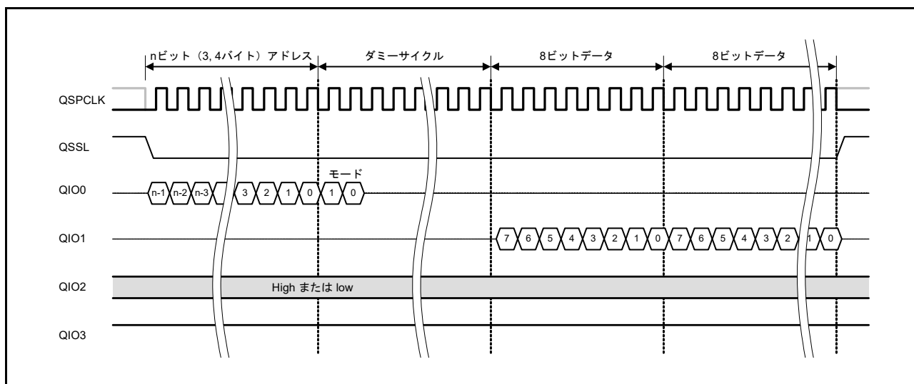
図 39.17 XIP モード時のファストリードバスサイクル
