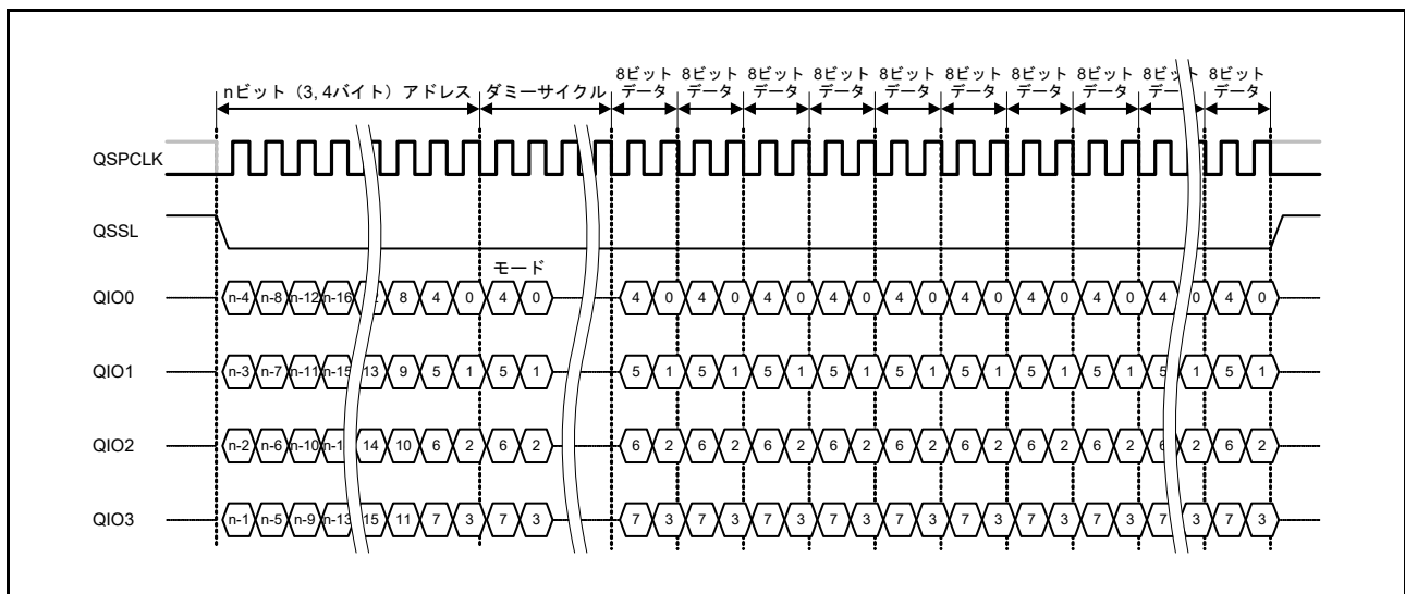
図 39.25 XIP モード時のファストリード Quad I/O バスサイクル
