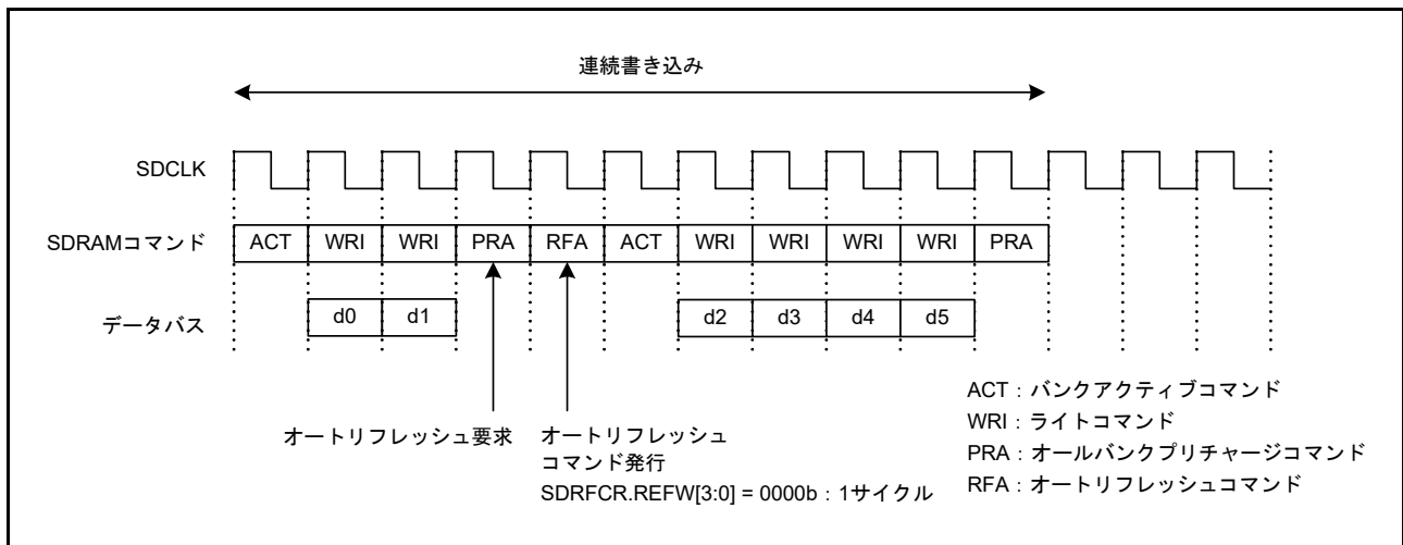
図 15.48 オートリフレッシュサイクルのタイミング例 (3) (連続アクセス中にオートリフレッシュ要求が発生した場合)
