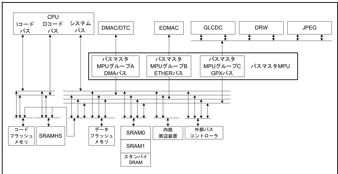
図 16.3 バスマスタ MPU ブロック図
