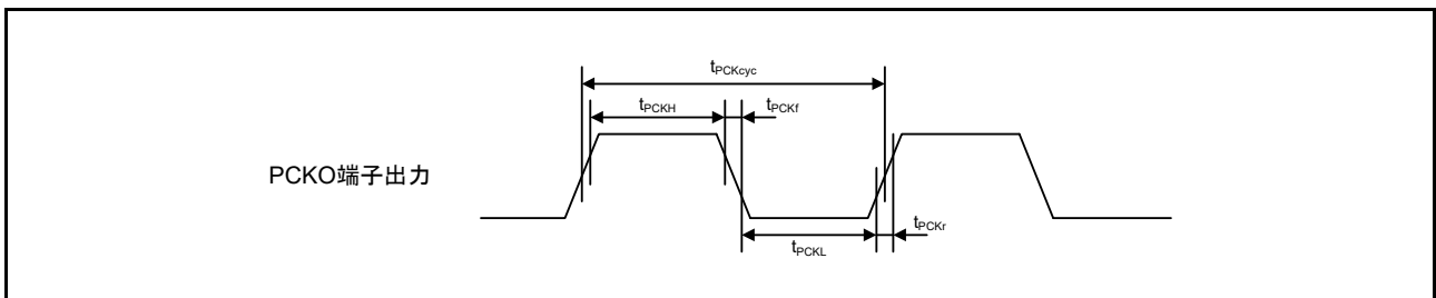
図 60.78 PDC 出力クロックタイミング
