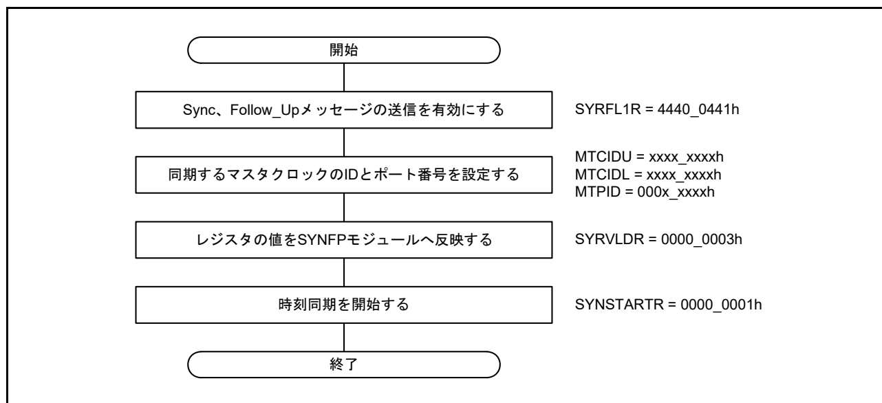
図 30.18 P2P スレーブ動作の開始手順
