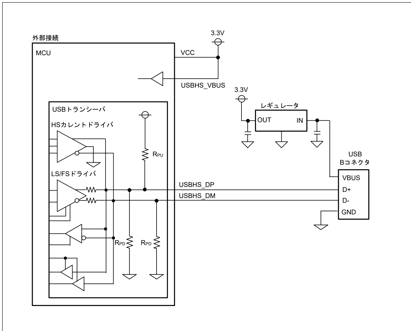
図 30.29 パスパワーシステムでのデバイス接続例
