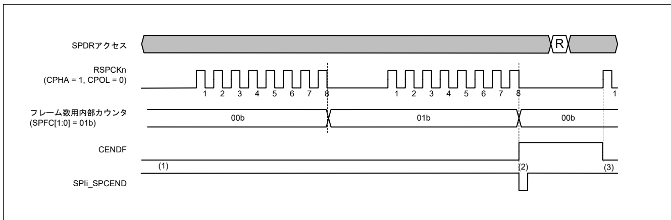
図 36.45 通信終了割り込み動作例 (クロック同期式動作時の受信のみスレーブモード)
