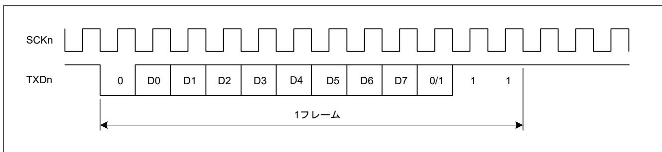
図 31.8 調歩同期式モードにおける出力クロックと送信データの位相関係 (CCR1.PE = 1、CCR3.CHR[1:0] = 10b、MP = 0、および STP = 1 の場合)
