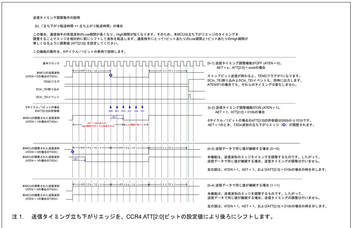
図 31.34 AET が 1 の場合の送信タイミング調節動作の説明
