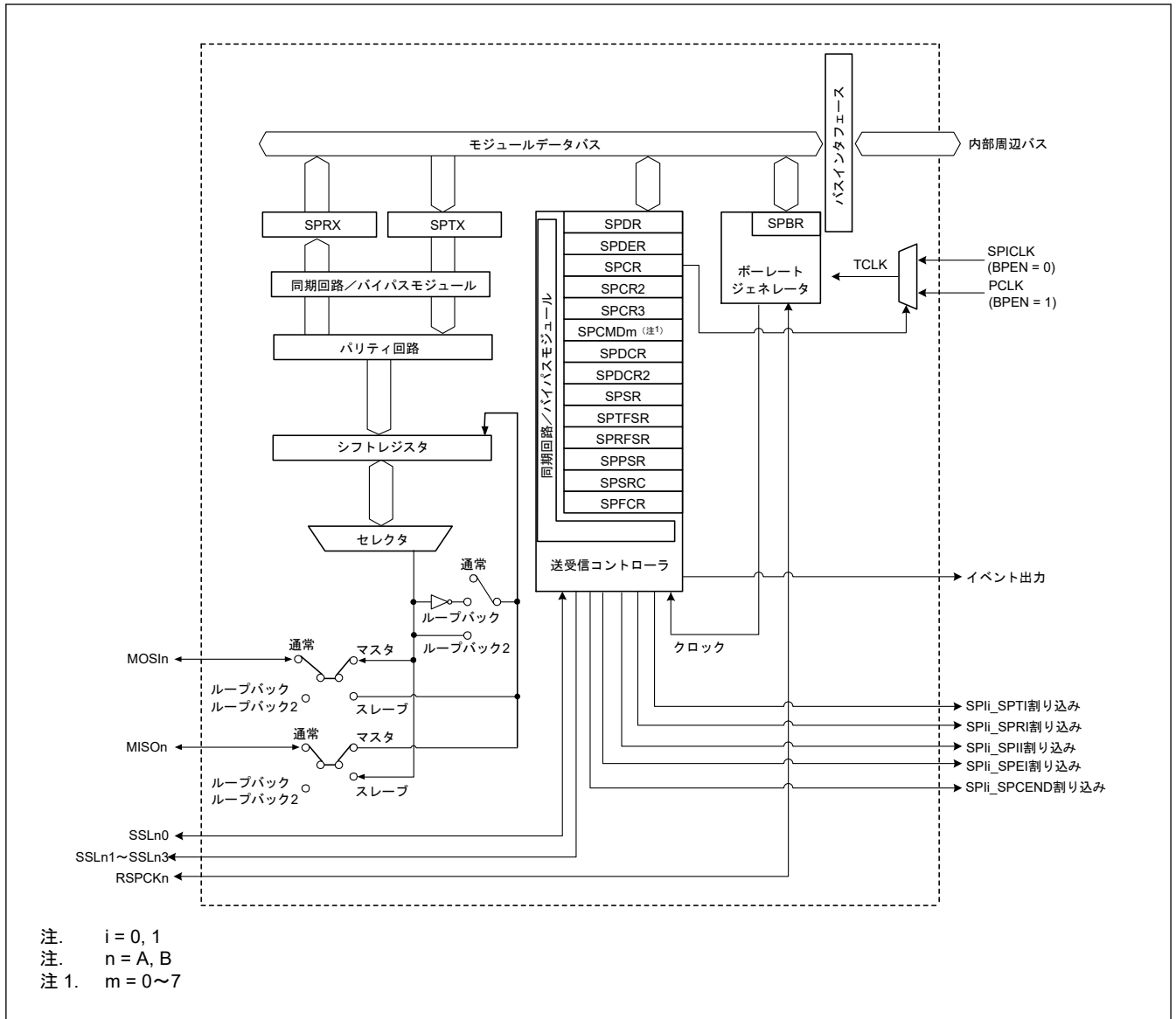
図 36.1 SPIのブロック図
