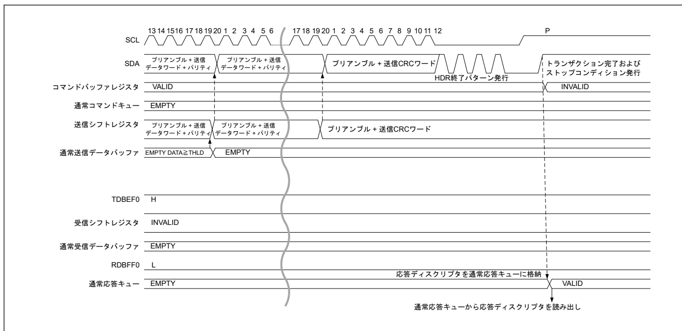
図 33.27 HDR データ書き込み転送 (HDR-DDR) タイミング (4/4)
