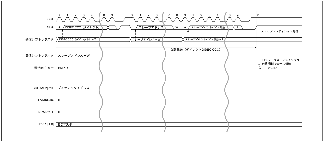
図 33.109 バス権要求 : NACK (DVMRRJ が 1) かつ NRMRCCTL が 1 の場合 (2/2)
