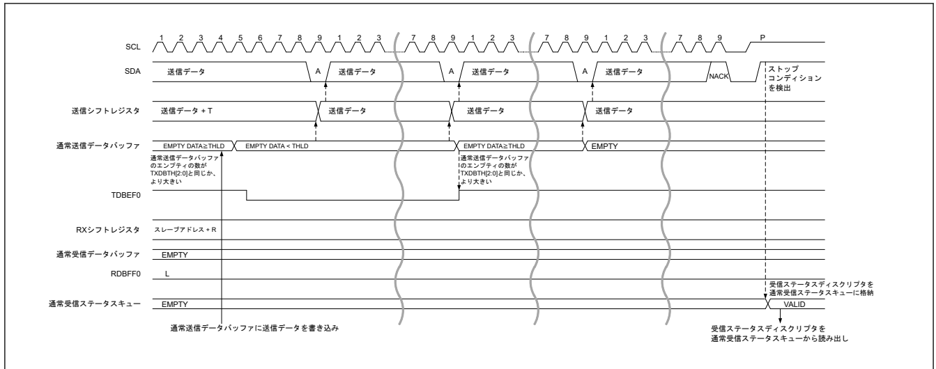
図 33.52 レガシー I 2 C メッセージデータ読み出し転送タイミング (2/2)
