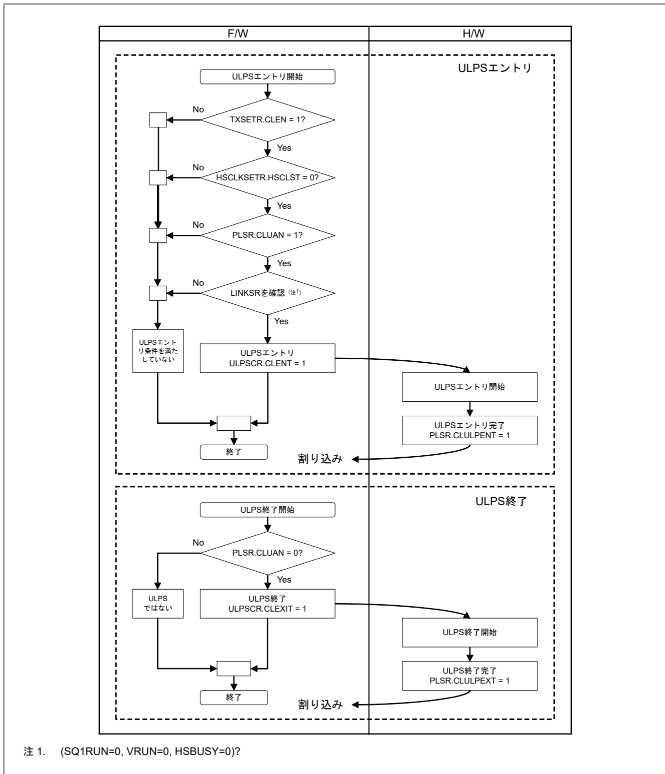
図 58.7 ULPS 遷移/復帰 (クロックレーン)
