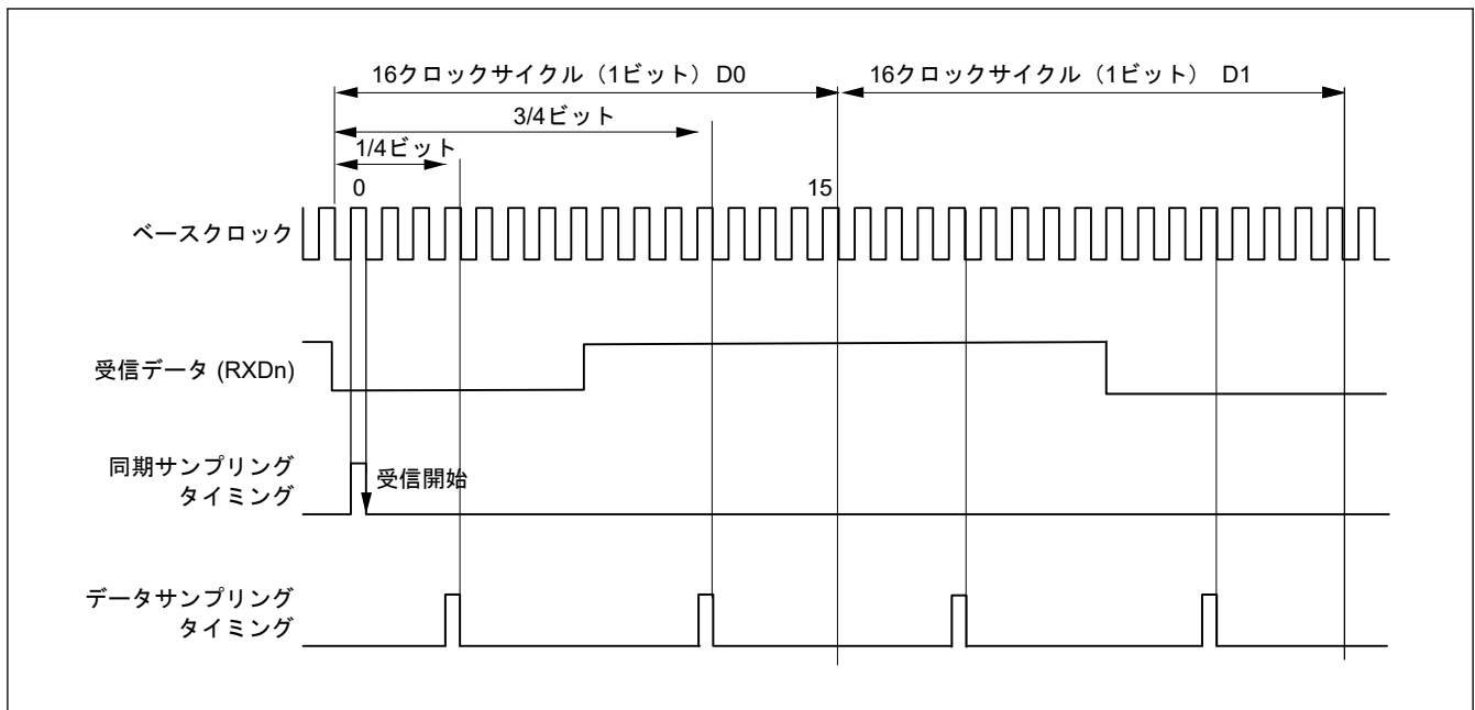
図 31.55 マンチェスタモードでのデータ受信サンプリングタイミング
