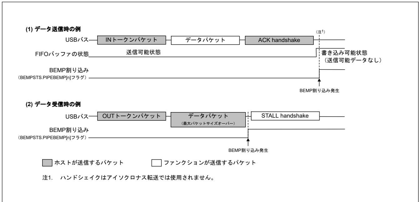
図 30.7 デバイスコントローラモード時の BEMP 割り込みの発生タイミング
