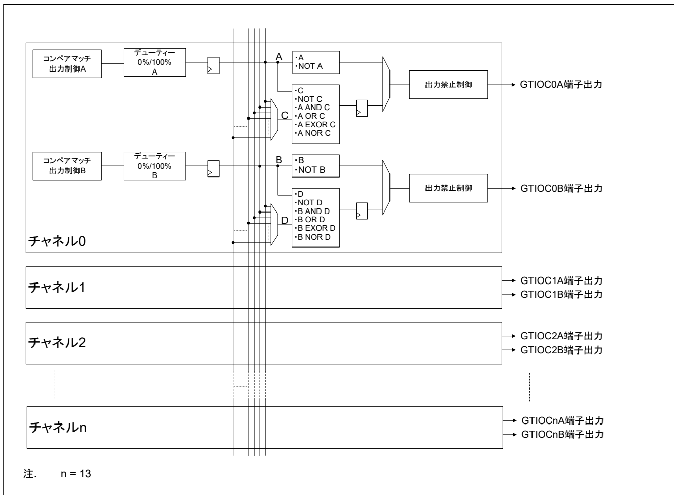
図 21.68 チャネル間論理演算のブロック図
