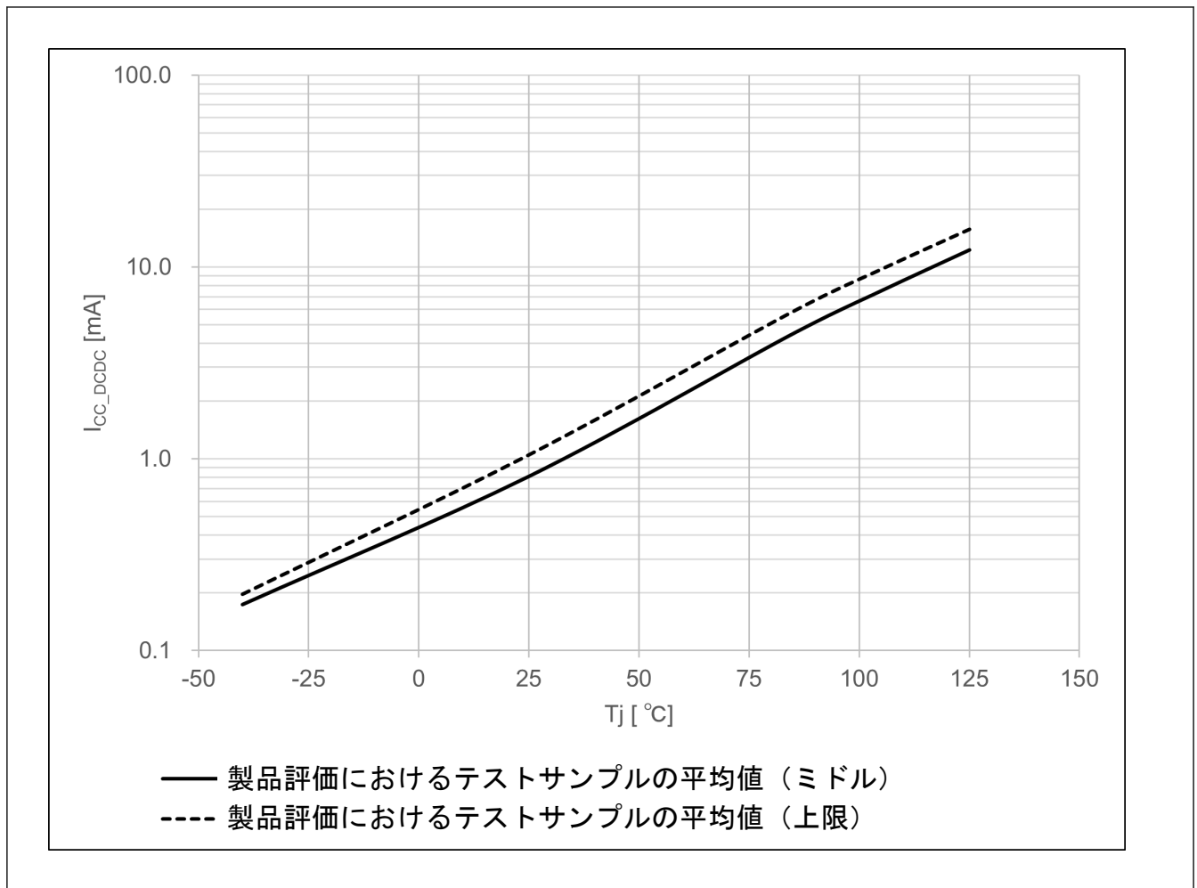
図 60.4 ソフトウェアスタンバイモードにおける温度依存性 ( I_{cc\_DCDC} ) (参考データ)
