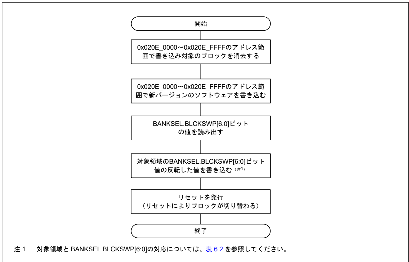
図 52.36 セキュアエイリアスのブロックスワップ選択フロー例 (2 MB のコードフラッシュメモリを持つ製品の場合)
