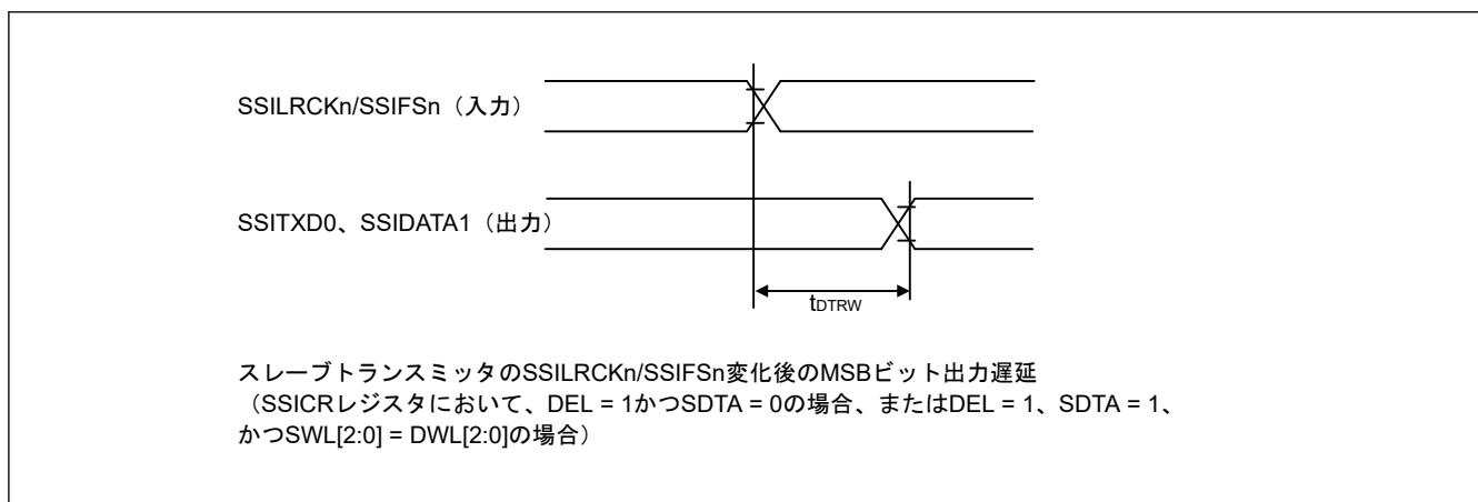
図 60.89 SSILRCK0/SSIF0 変化時からの SSIE データ出力遅延
