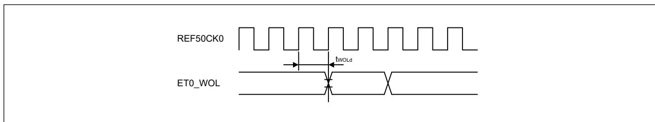
図 60.95 RMII に対する WOL 出力タイミング
