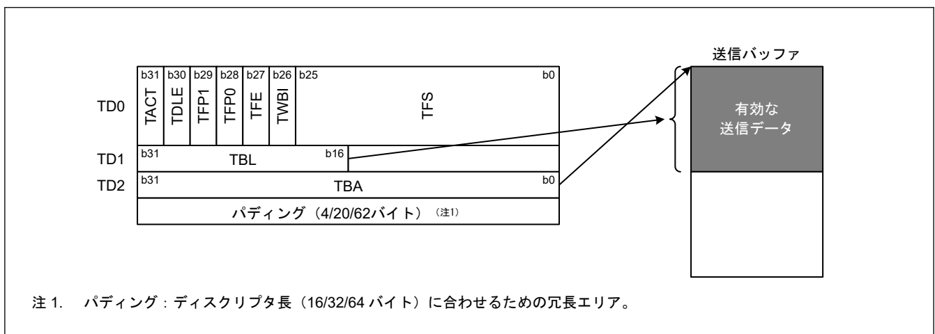
図 28.3 送信ディスクリプタと送信バッファの関係
