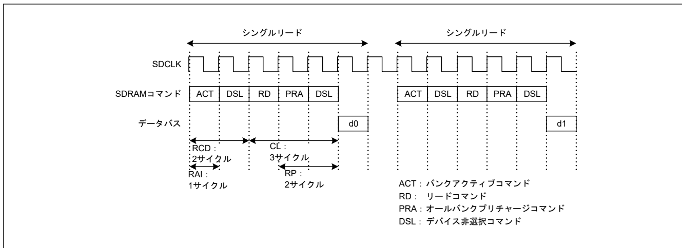
図 14.54 シングルリードタイミング例 (3)
