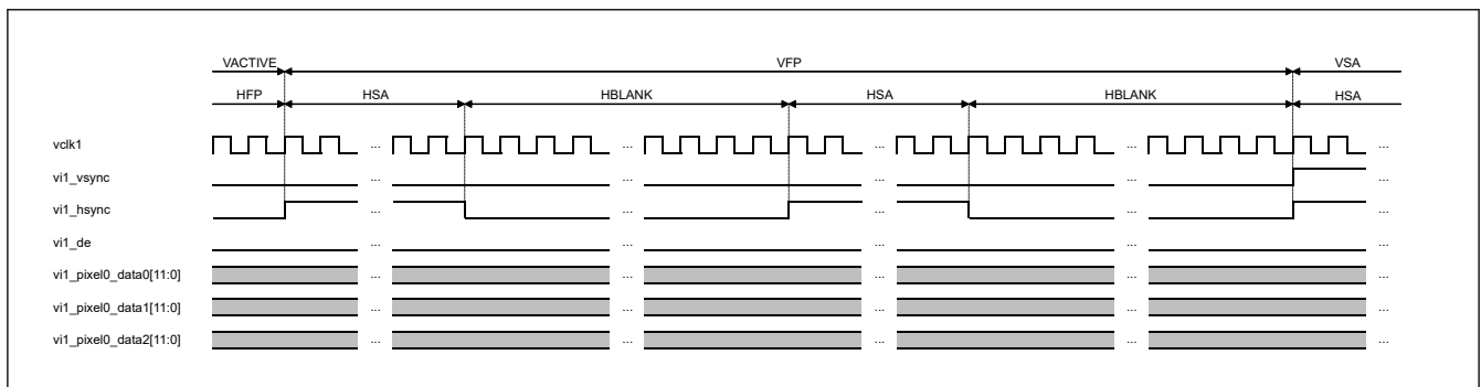
図 58.14 VACTIVE 終了および VFP 開始
