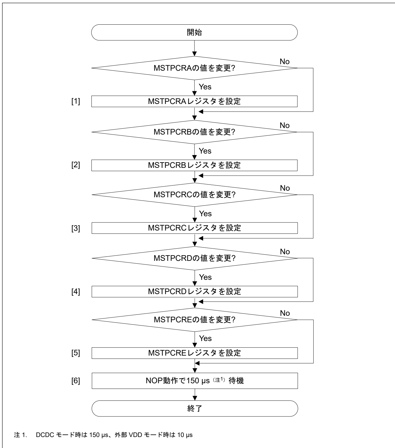
図 10.2 CPUCLK が 120 MHz より高い場合のモジュールストップコントロールレジスタの設定フロー
