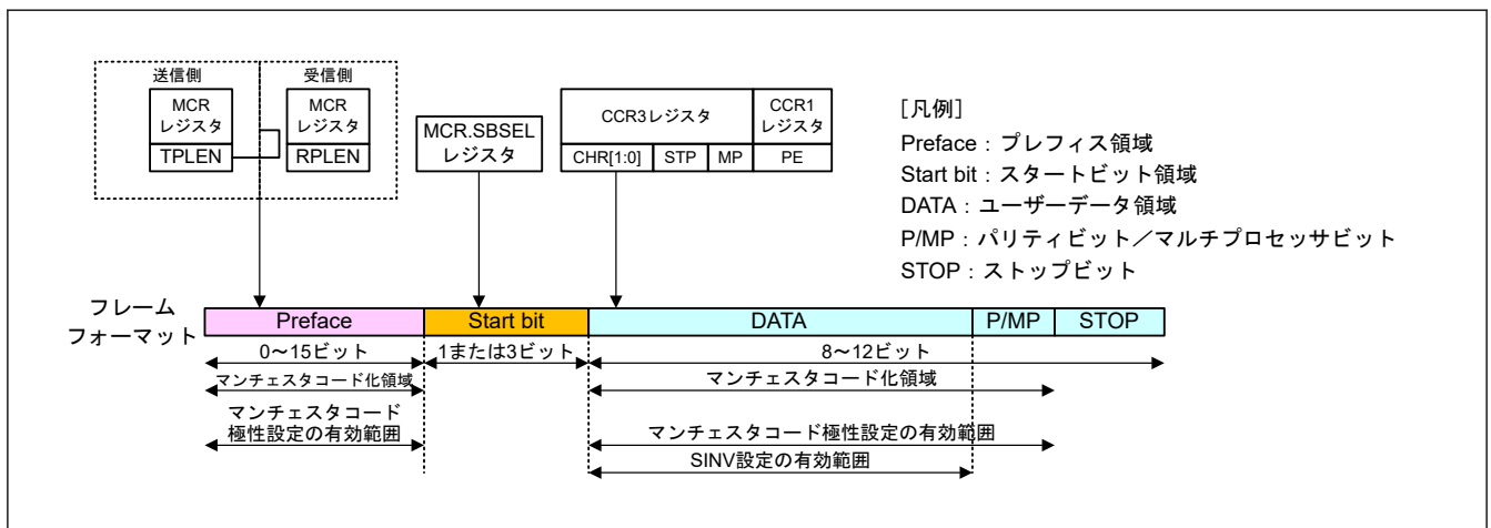
図 31.46 マンチェスタモードでのフレームフォーマット
