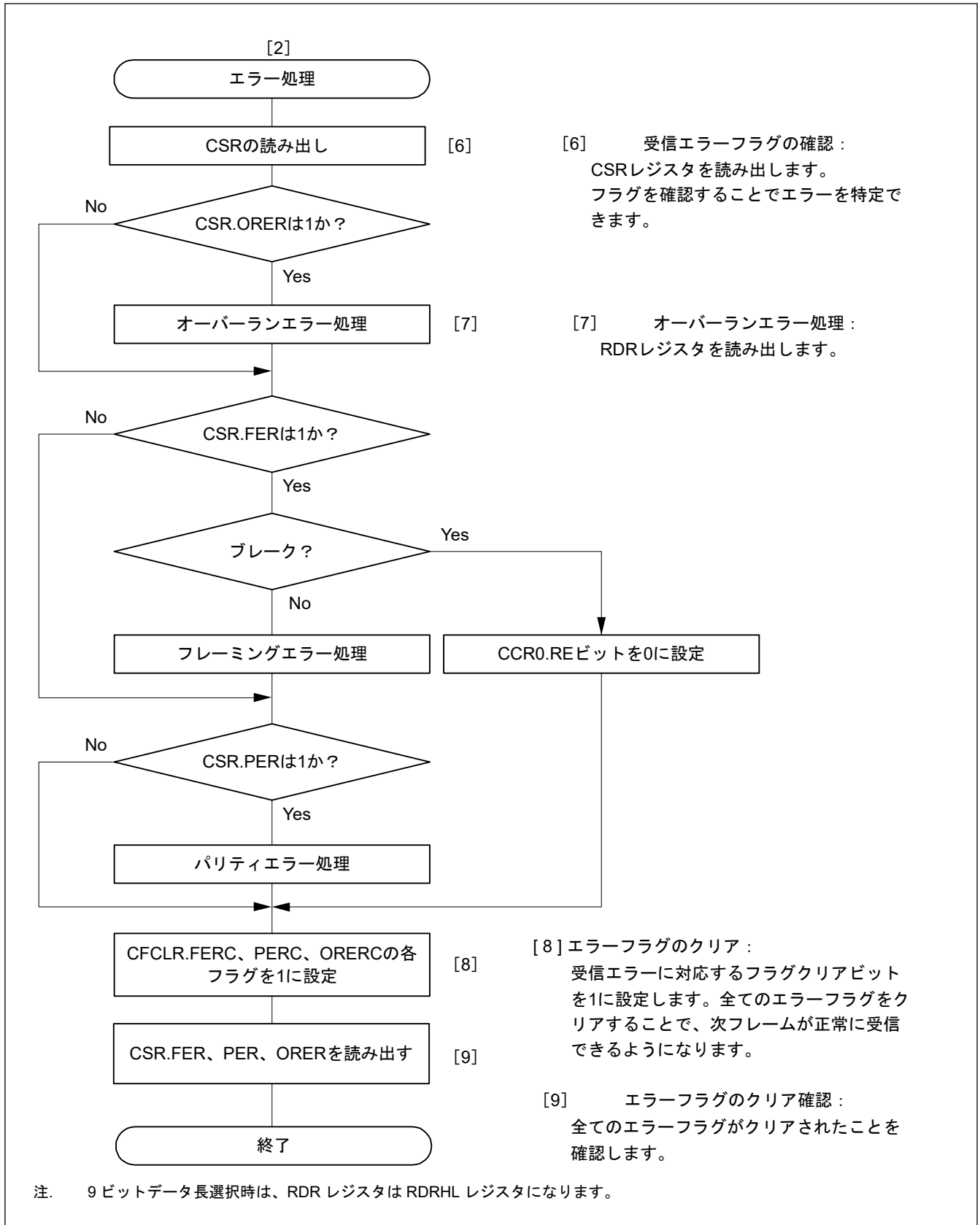
図 31.22 調歩同期式モードにおけるシリアル受信のフローチャート例（非 FIFO 選択、アドレス一致検出無効時）(2)
