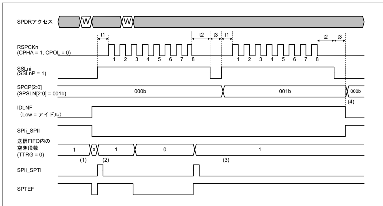
図 36.34 アイドル割り込み動作の例 (マスタモード/Motorola-SPI)
