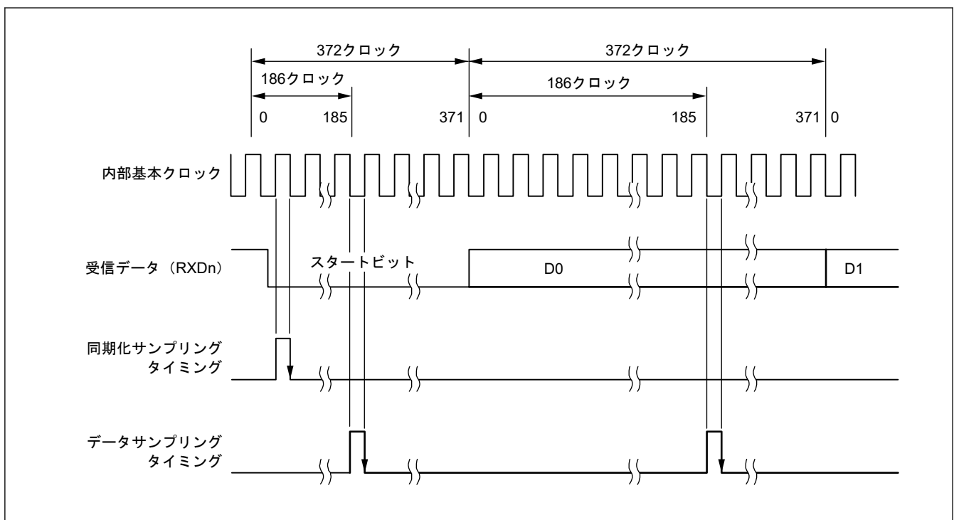
図 31.78 スマートカードインタフェースモードにおける受信データのサンプリングタイミング（ビットレートの 372 倍のクロック周波数の場合）
