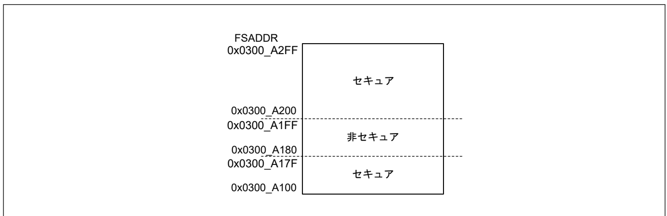
図 52.41 オプション設定メモリ内のセキュア領域と非セキュア領域 (セキュアエアリアスの場合)
