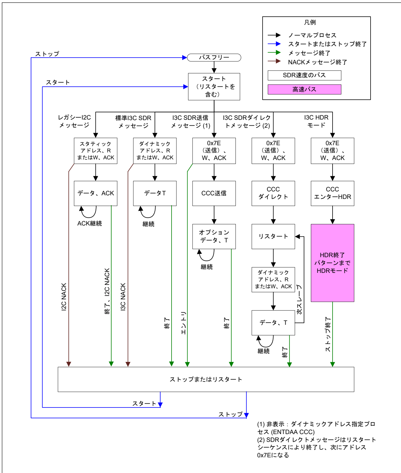
図 33.142 I3C 通信フロー
