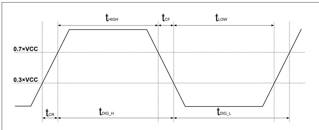
図 60.74 t_{DIG\_H} 、 t_{DIG\_L}
