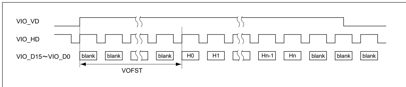
図 53.17 垂直オフセット
