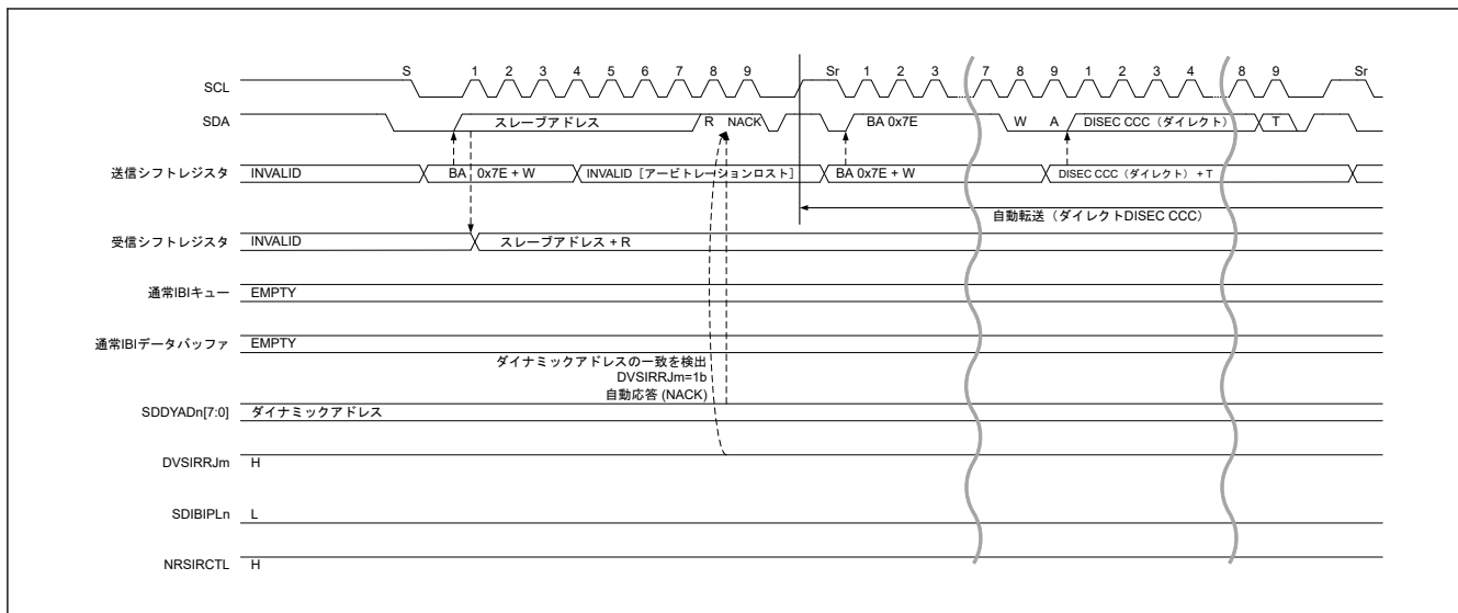
図 33.103 スレーブ割り込み要求 : NACK (DVSIRRJ が 1) かつ NRSIRCTL が 1 の場合 (1/2)
