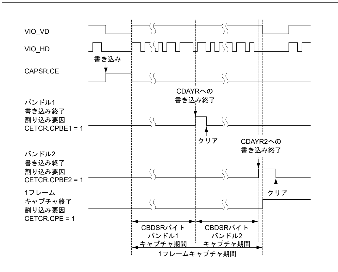
図 53.43 書き込み終了割り込みのタイミング (データイネーブル取り込み時)
