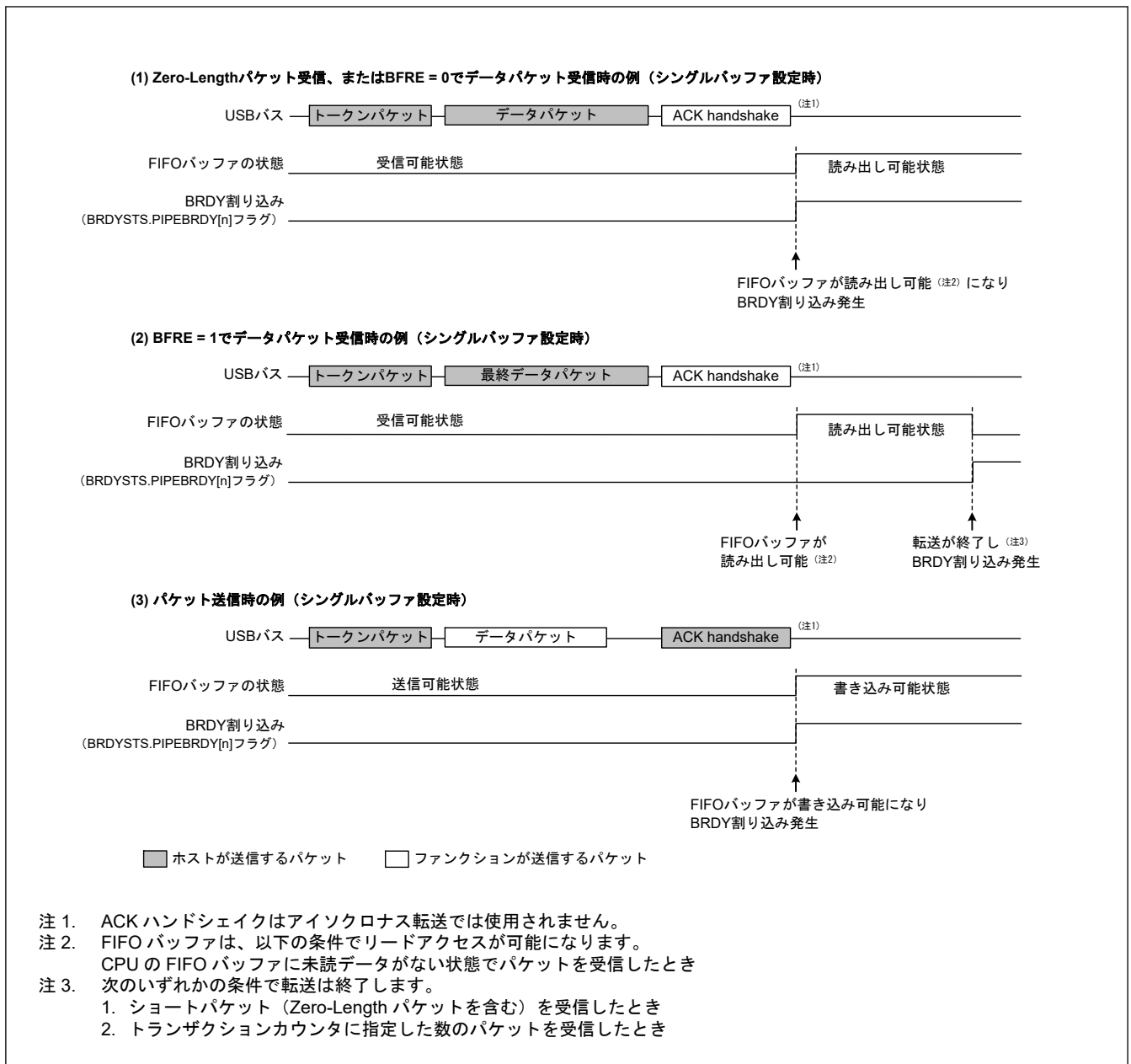
図 30.5 BRDY 割り込み発生タイミング
