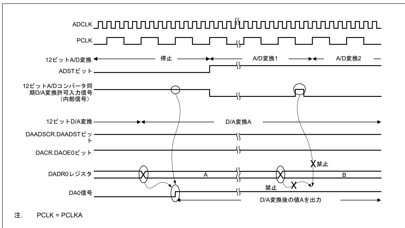
図 46.4 DAC12 が次からの同期 D/A 変換許可入力信号を取り込めない場合の例：ADC12 (ユニット 1)
