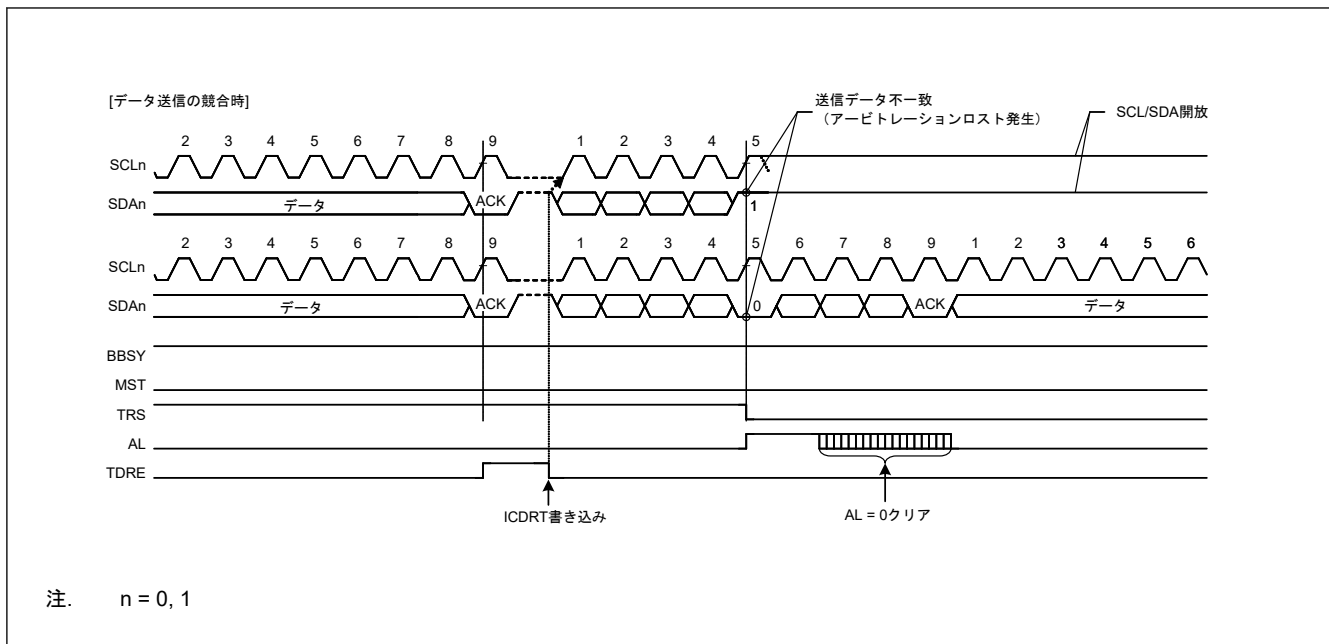
図 32.44 スレーブアービトラージョンロスト検出動作例 (SALE = 1 の場合)
