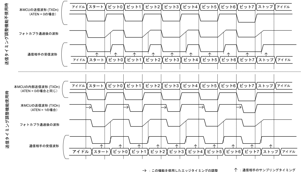
図 31.32 フォトカプラを経由する送信波形の説明
