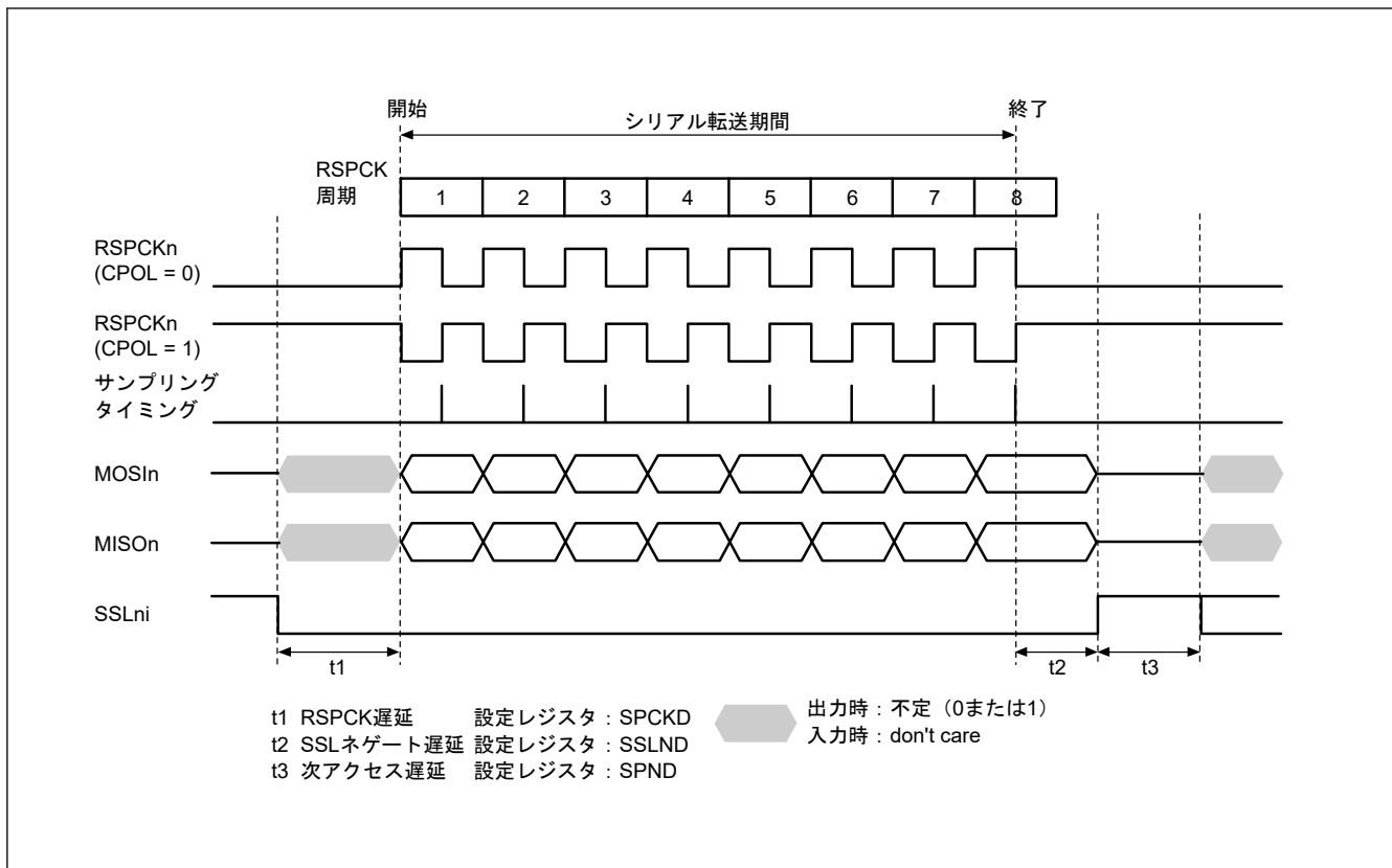
図 36.28 SPI 転送フォーマット (CPHA = 1、SPFRF = 0 の場合)
