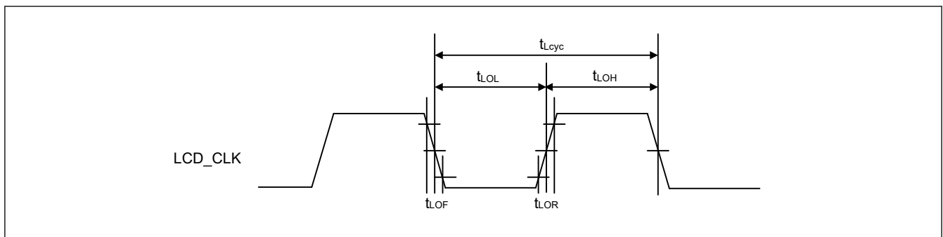
図 60.104 LCD_CLK クロック出力タイミング
