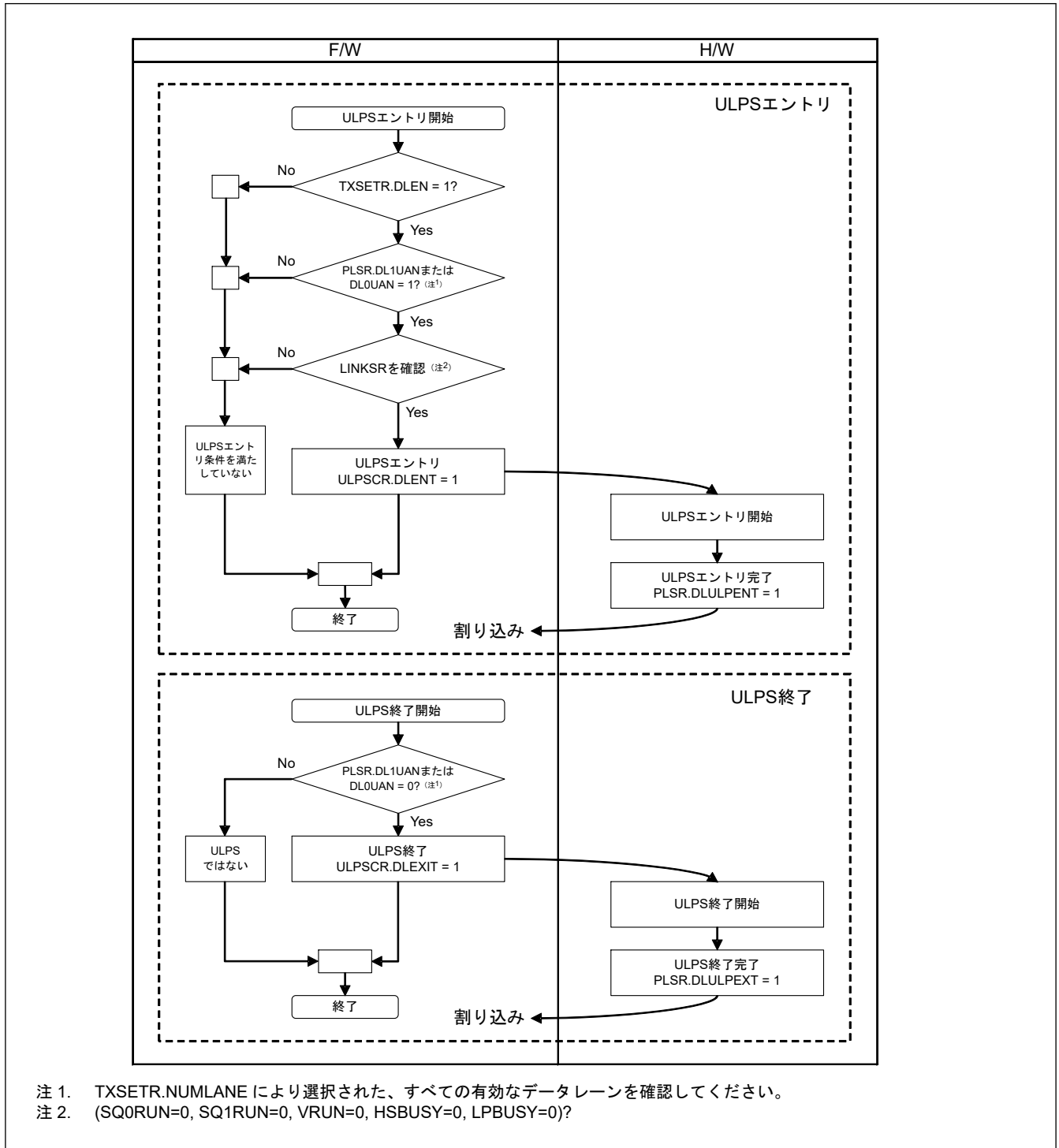
図 58.6 ULPS 遷移/復帰 (データレーン)
