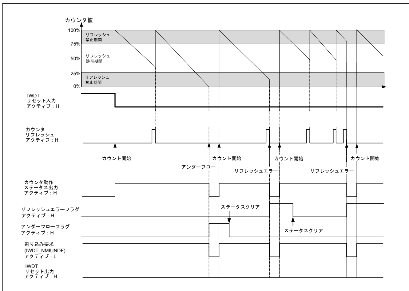
図 26.4 オートスタートモードでの動作例
