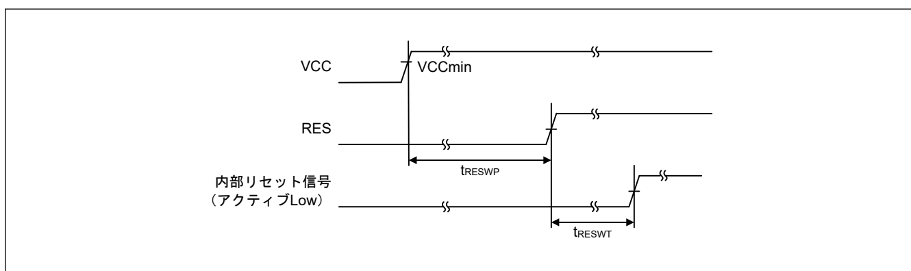
図 60.22 VCC が VPPOR 電圧しきい値を超える条件下での RES 端子入カタイミング
