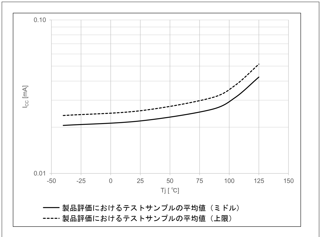
図 60.3 ソフトウェアスタンバイモードにおける温度依存性 ( I_{cc} ) (参考データ)
