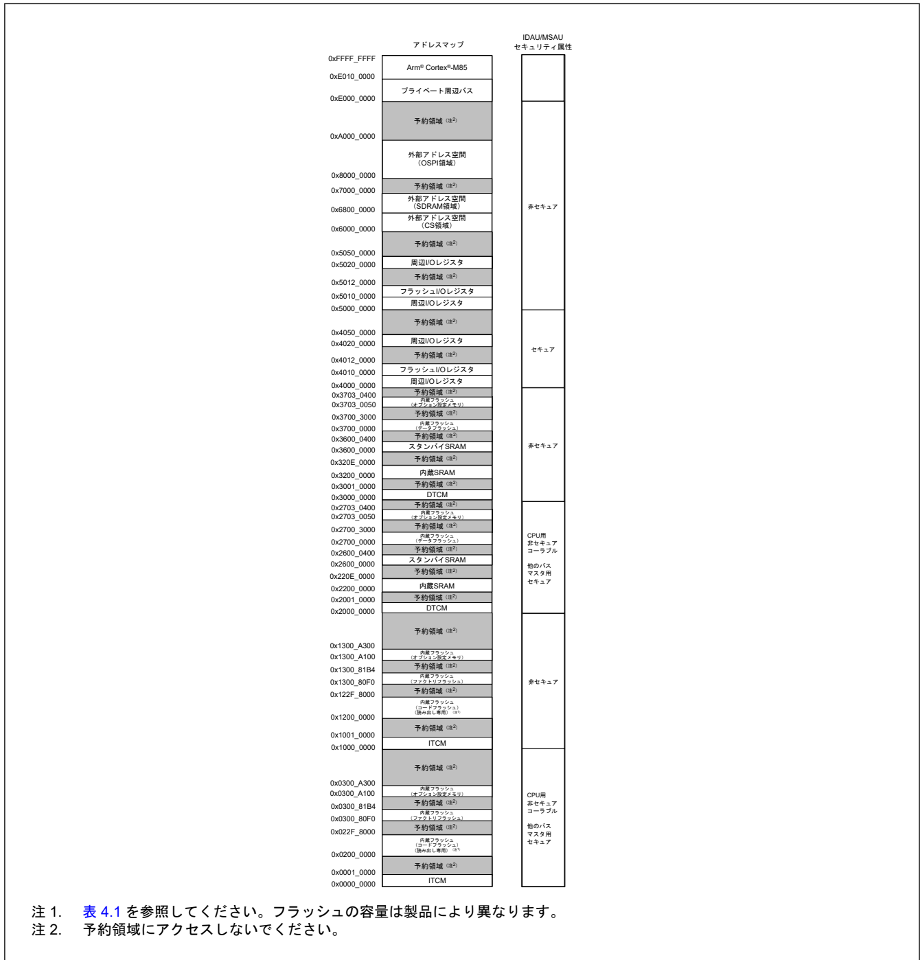
図 4.1 2 MB のフラッシュ製品のメモリマップの例
