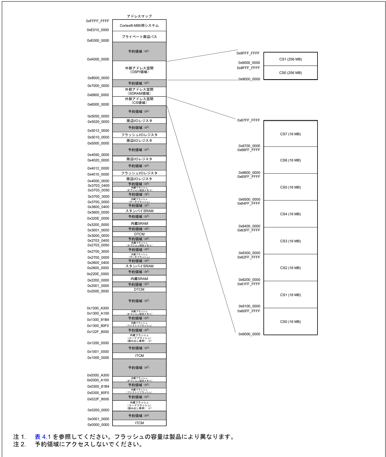
図 4.2 CS 領域と OSPI 領域のアドレスマップの詳細
