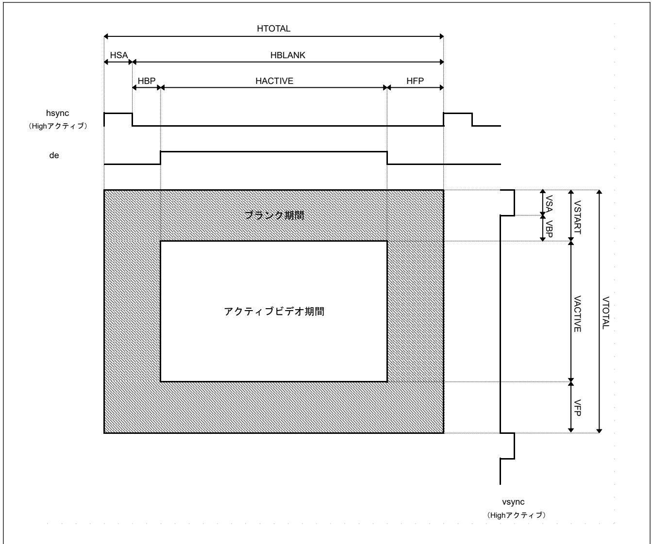
図 58.9 ビデオモードのタイミング
