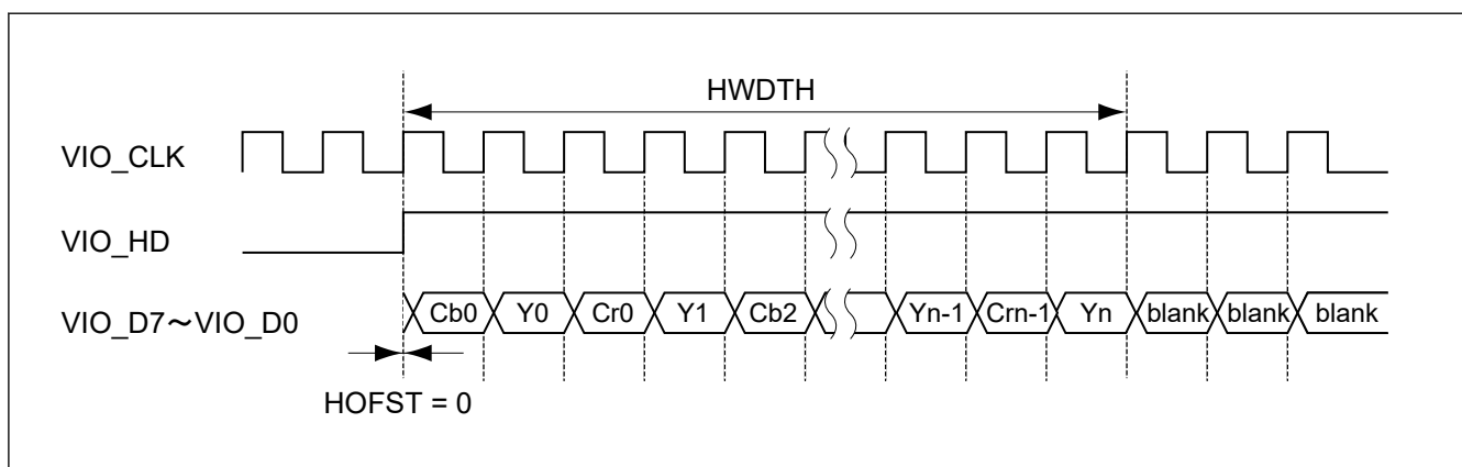
図 53.22 水平キャプチャタイミング (画像キャプチャ 8 ビットインターフェース)
