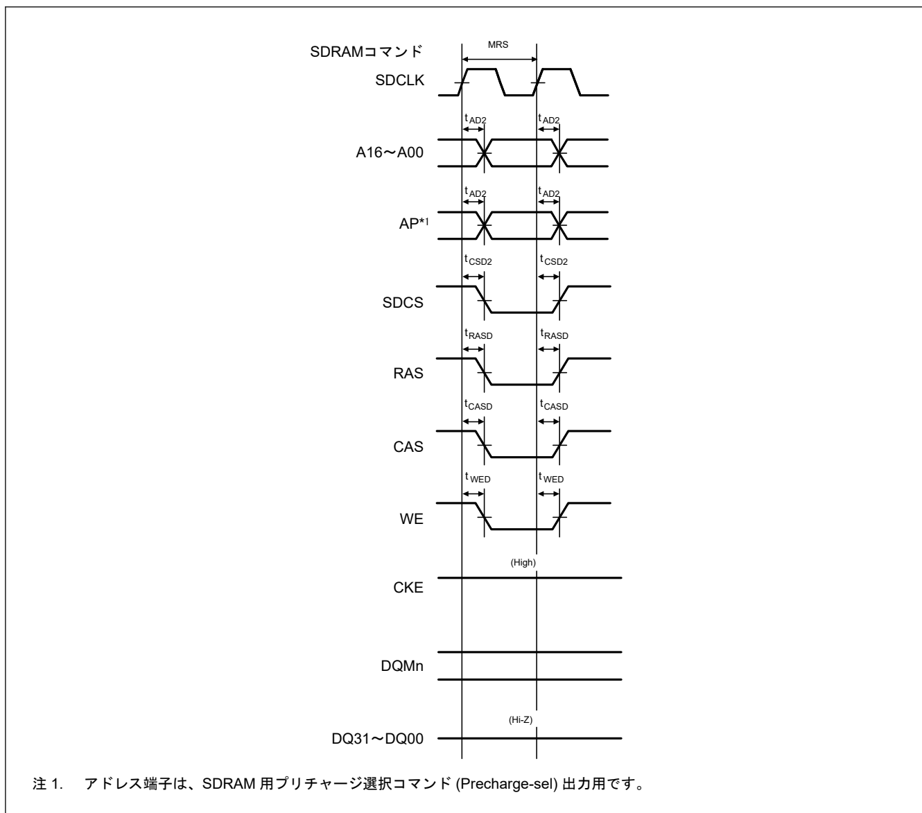
図 60.40 SDRAM モードレジスタの設定のタイミング
