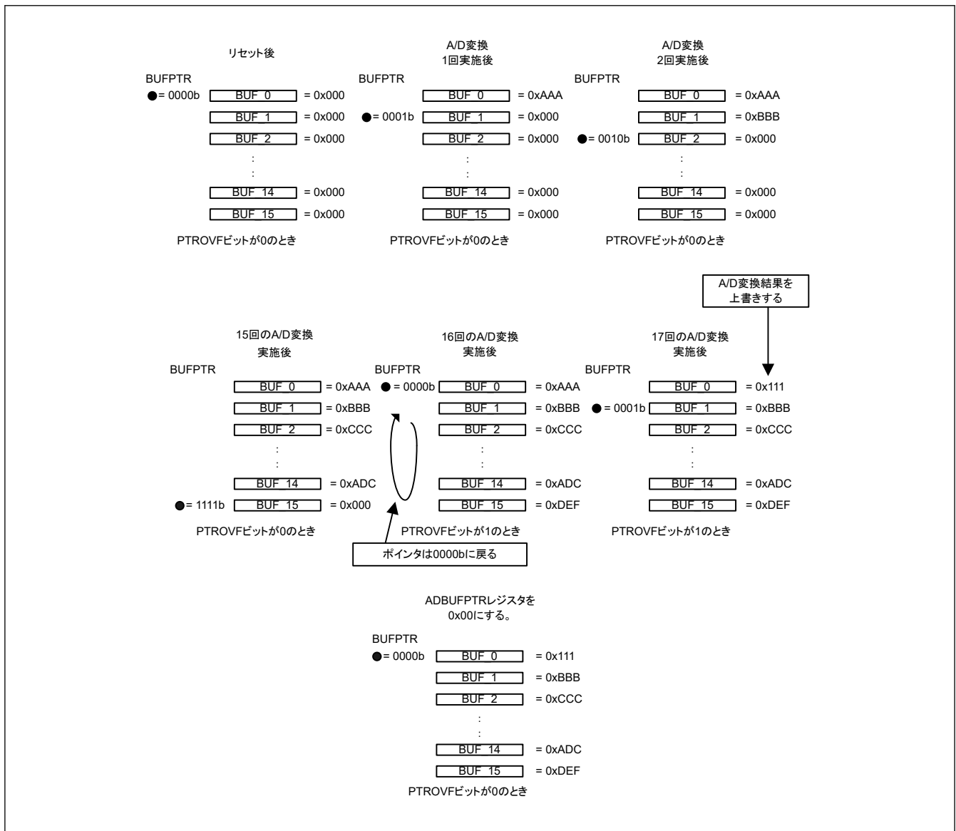
図 45.42 データバッファ、ポインタ、およびオーバーフローフラグの動作概略図
