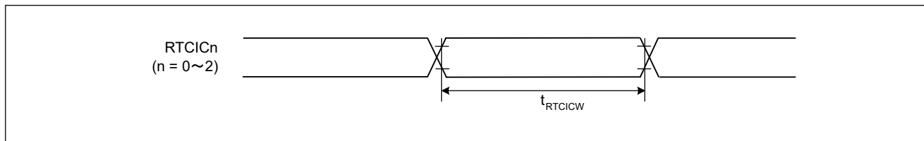
図 60.43 RTCICn 入カタイミング
