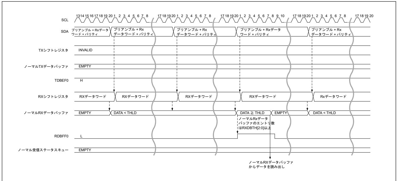
図 33.54 HDR データ書き込み転送 (HDR-DDR) タイミング (2/3)
