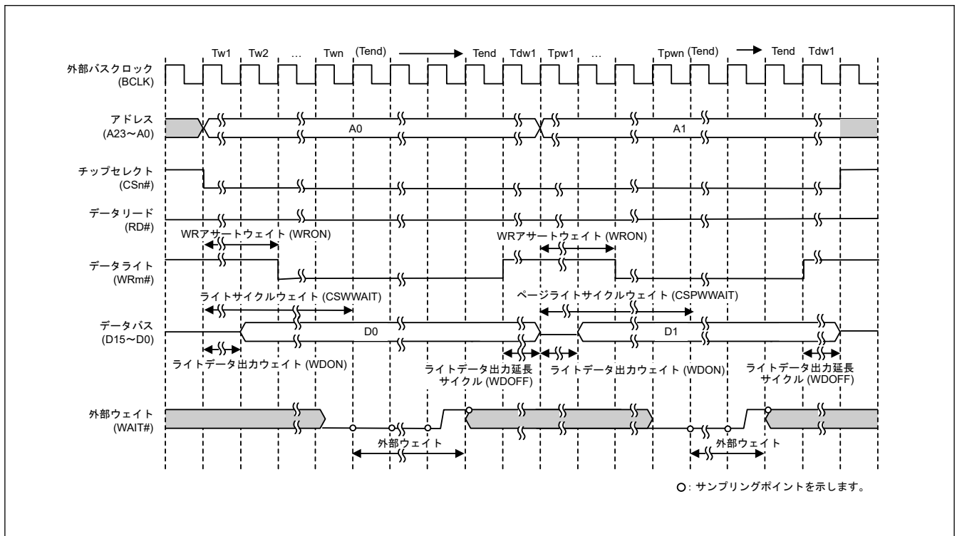
図 14.26 外部ウェイトタイミング例 (バイトストローブモード時の 16 ビットバス空間に対するページライトアクセス、BCLK 端子出力選択ビットで BCLK の 1 分周を選択した場合) (n = 0~7, m = 0, 1)
