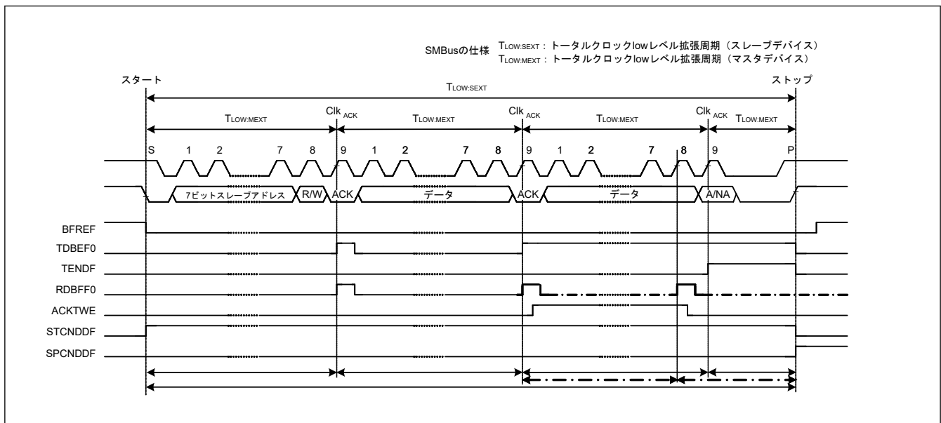
図 33.114 SMBus タイムアウト測定
