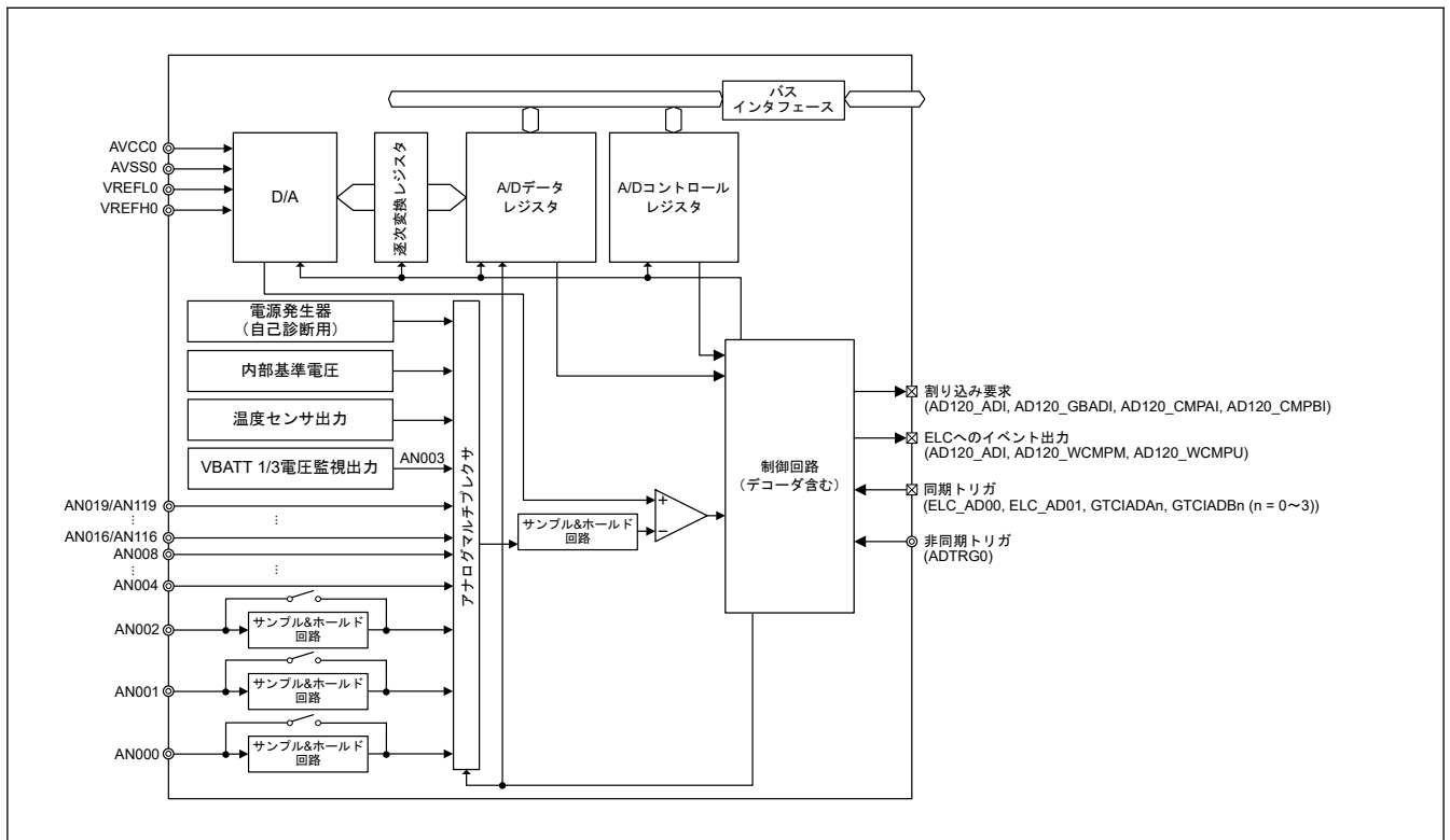
図 45.1 ADC12 ブロック図 (ユニット 0)
