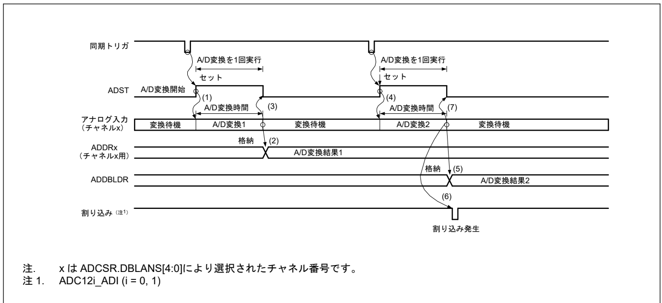
図 45.15 シングルスキャンモードの動作例 (ダブルトリガモード選択、アナログ入力 (チャンネル x) を 2 重化)
