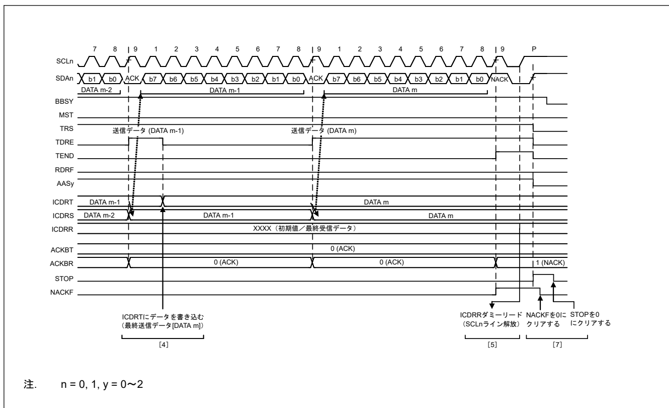
図 32.17 スレーブ送信の動作タイミング (2)
