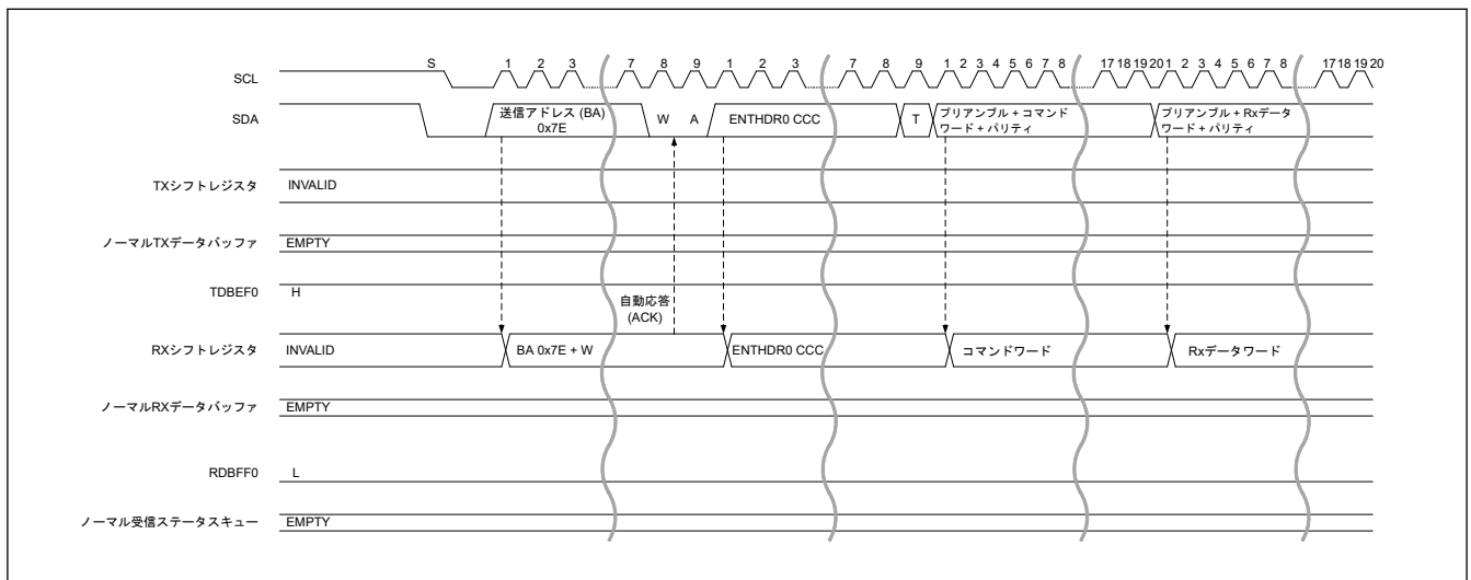
図 33.53 HDR データ書き込み転送 (HDR-DDR) タイミング (1/3)
