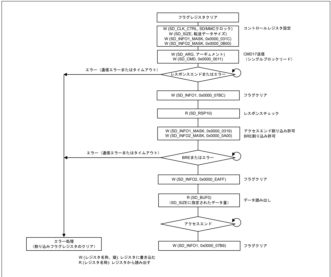
図 40.11 シングルブロックリード動作のフロー例
