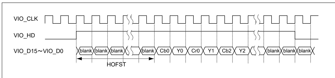
図 53.19 水平オフセット
