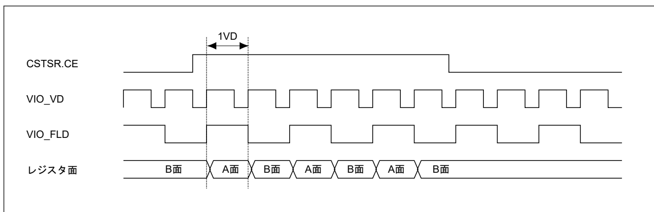
図 53.31 RVS = 1 のときのレジスタ面切り替えタイミング
