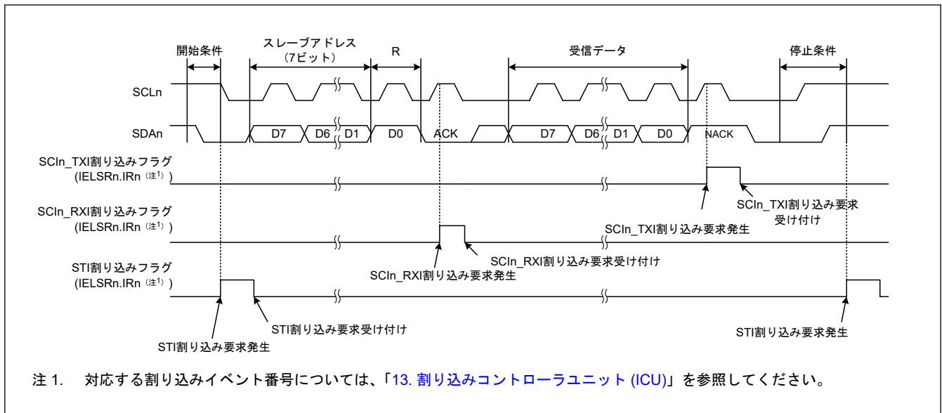
図 31.95 簡易 IIC モードにおけるマスタ受信の動作例 (7 ビットスレーブアドレス、ACK 割り込み、NACK 割り込み使用時) (ICR.IICINTM = 0)
