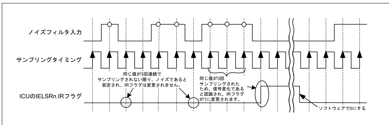
図 48.5 ノイズフィルタおよび割り込み動作の例
