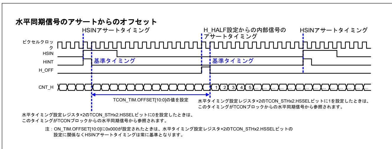
図 56.15 TCON 内水平同期信号生成用参照タイミング
