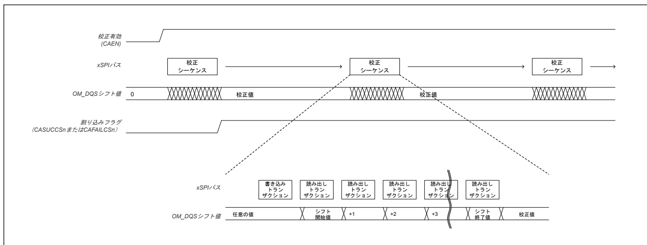
図 37.11 自動校正
