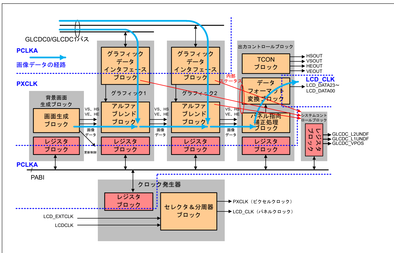
図 56.22 GLCDC の構成
