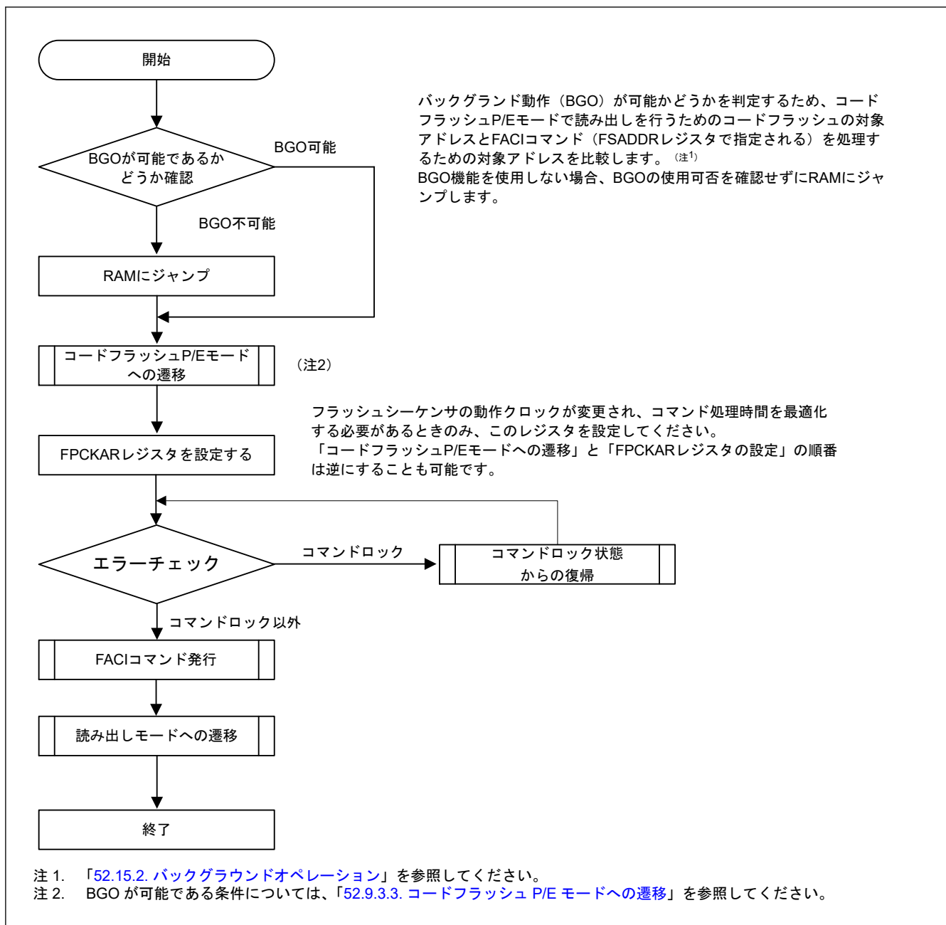
図 52.8 コードフラッシュ P/E モードでのコマンド使用概要
