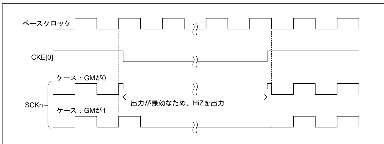
図 31.85 クロック出力タイミング
