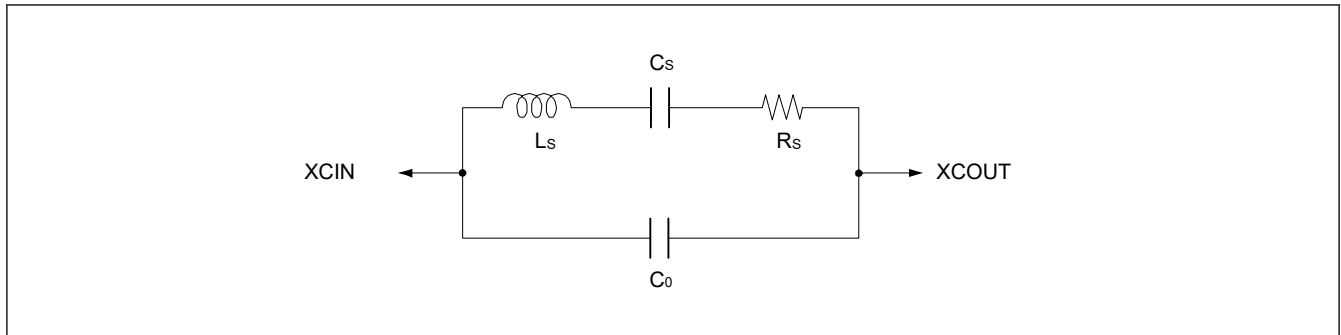
図 8.6 32.768 kHz 水晶振動子の等価回路
