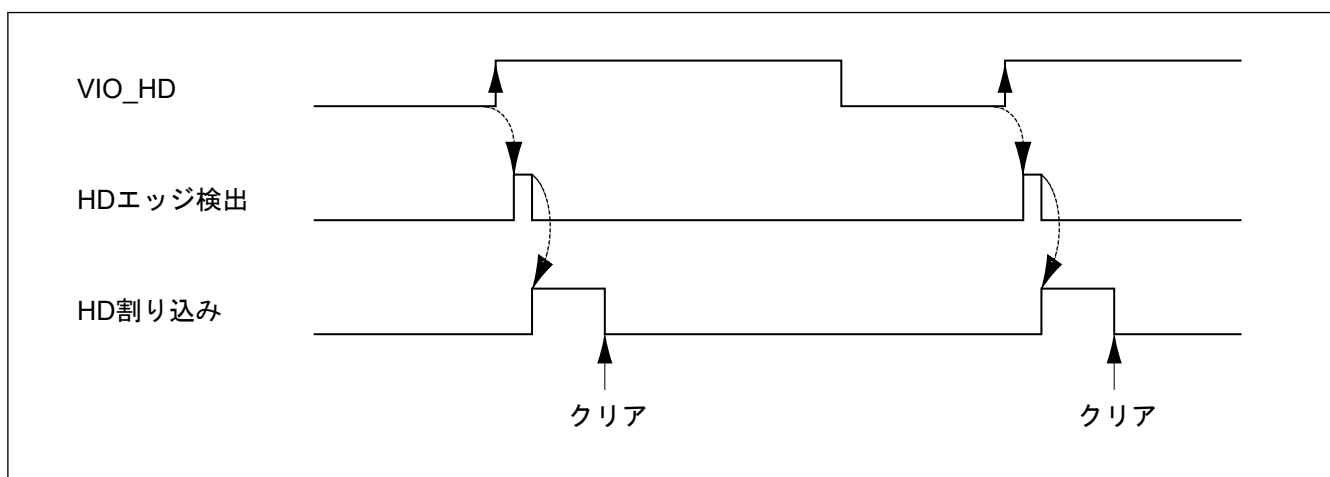
図 53.16 HD が正極性の場合の VIO_HD と HD 割り込みの関係
