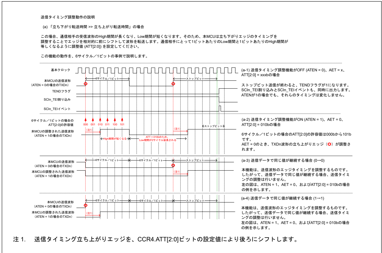
図 31.33 AET が 0 の場合の送信タイミング調節動作の説明
