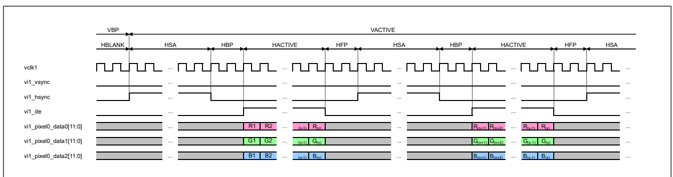
図 58.12 VBP 終了および VACTIVE 開始 (RGB)
