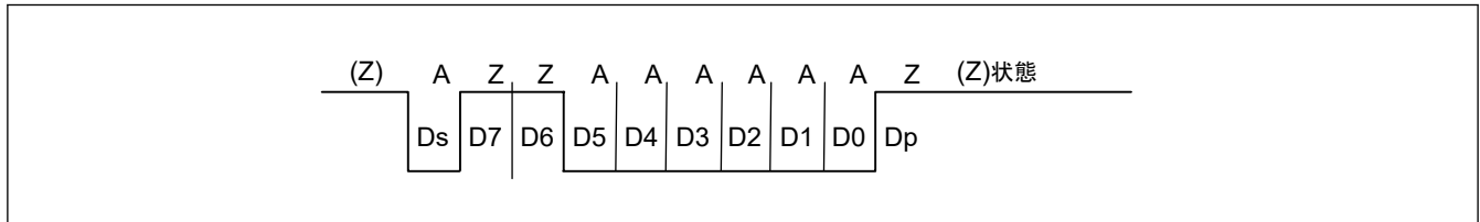
図 31.77 インバースコンベンション (CCR3.LSBF = 0、CCR3.SINV = 1、CCR1.PM = 1)
