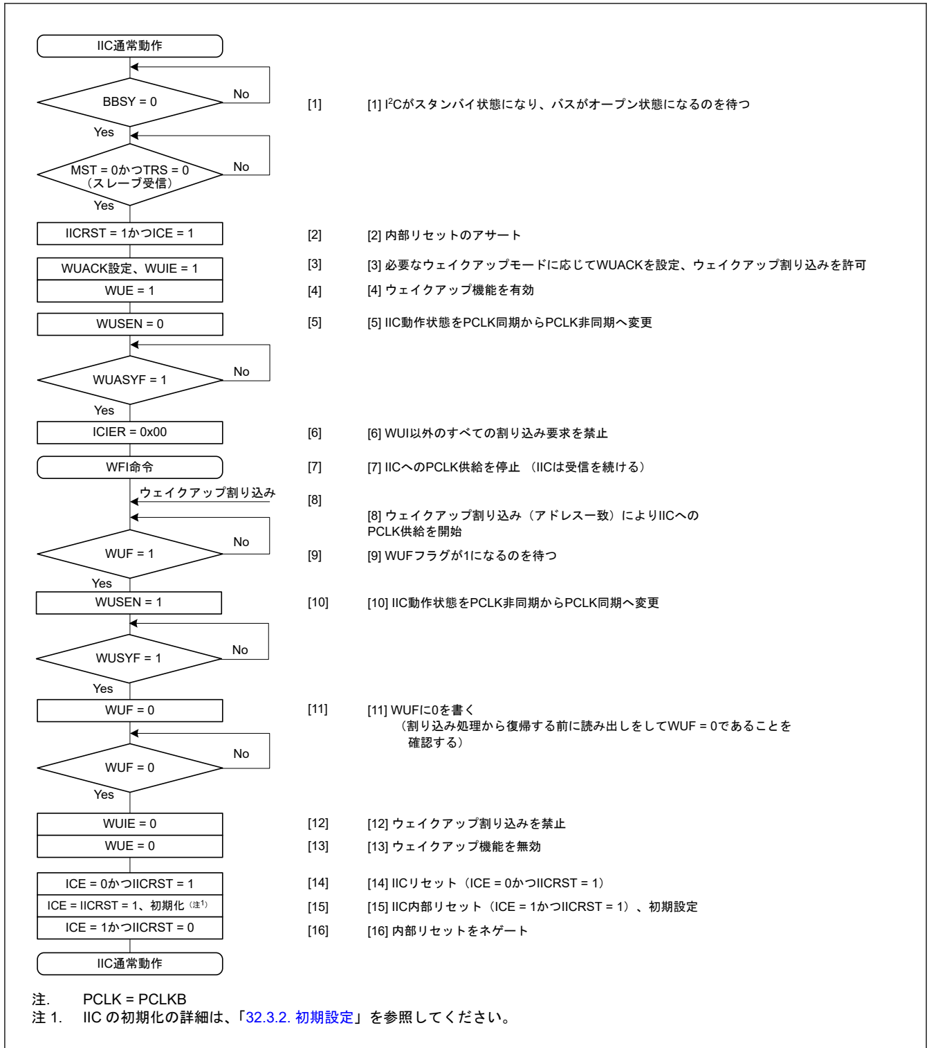
図 32.35 コマンドリカバリモードと EEP 応答モードの動作例 (スリープアドレス一致時のウェイクアップ割り込みによるウェイクアップの場合)
