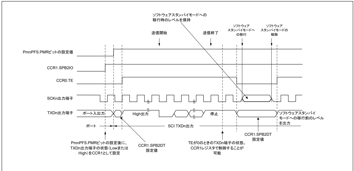
図 31.118 ソフトウェアスタンバイモード遷移時のポートの端子状態 (内部クロック、調歩同期送信)
