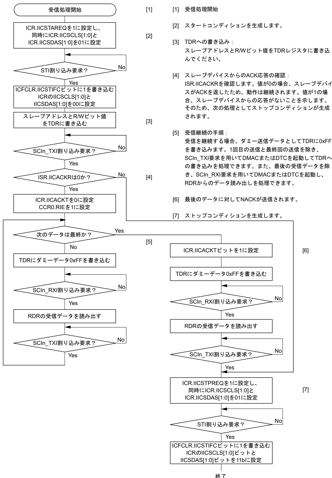
図 31.96 簡易 IIC モードにおけるマスタ受信のフロー例 (送信割り込み、受信割り込み使用時 (ICR.IICINTM = 1))
