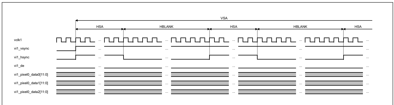
図 58.10 VSA 開始 (および VFP 終了)
