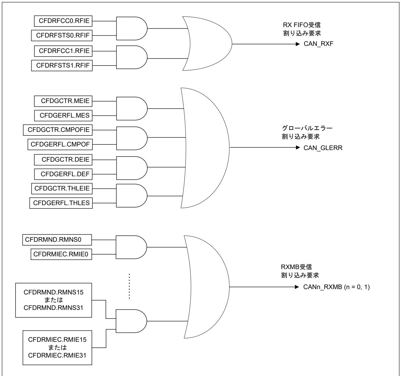
図 34.30 グローバル割り込みのブロック図
