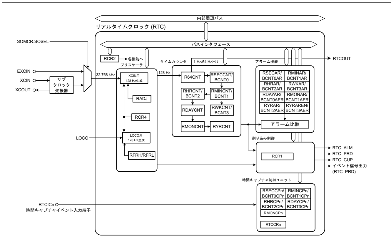
図 24.1 RTC のブロック図
