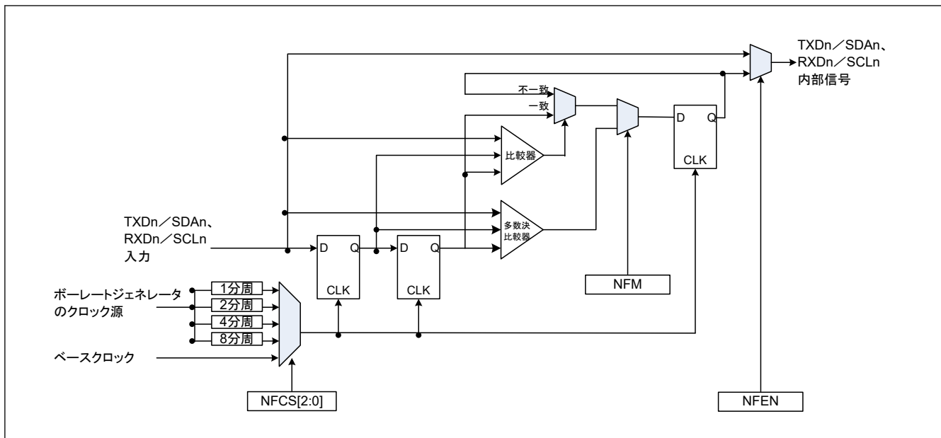
図 31.113 デジタルノイズフィルタ回路のブロック図
