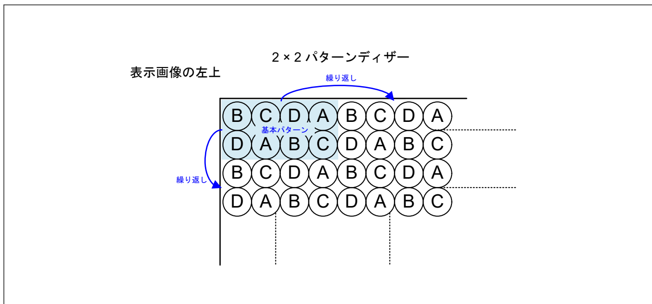
図 56.14 2x2 パターンディザーの加算値選択方式
