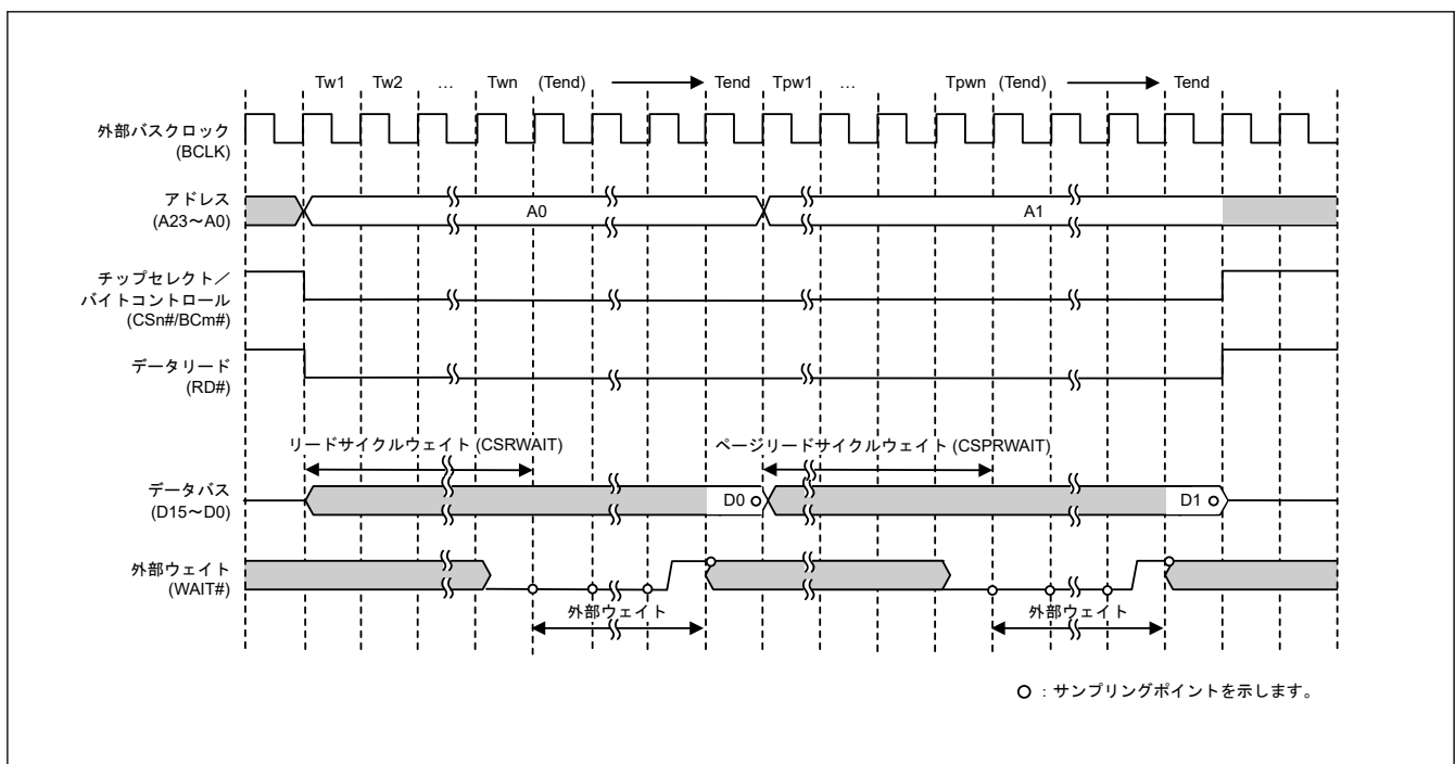
図 14.24 外部ウェイトタイミング例 (16 ビットバス空間に対するページリードアクセス、BCLK 端子出力選択ビットで BCLK の 1 分周を選択した場合) ( n = 0 \sim 7, m = 0, 1 )
