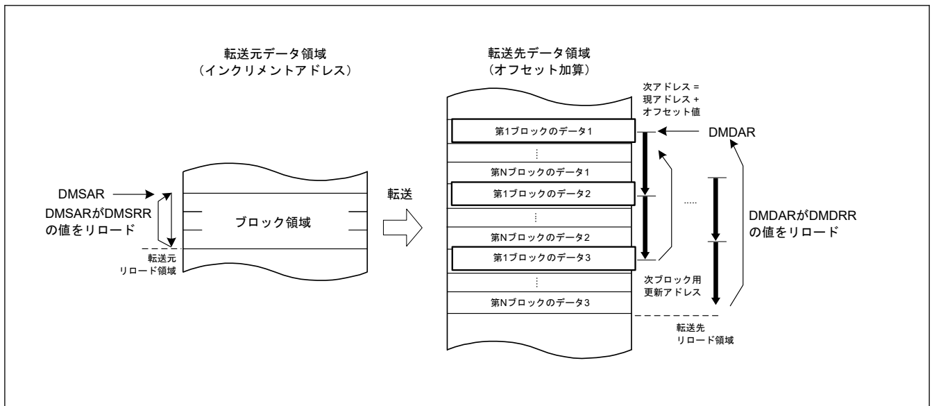
図 16.6 リピートブロック転送モードの動作 (オフセット加算)
