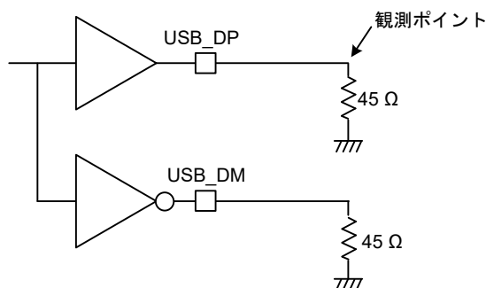
図 60.118 High-speed モードにおける測定回路
