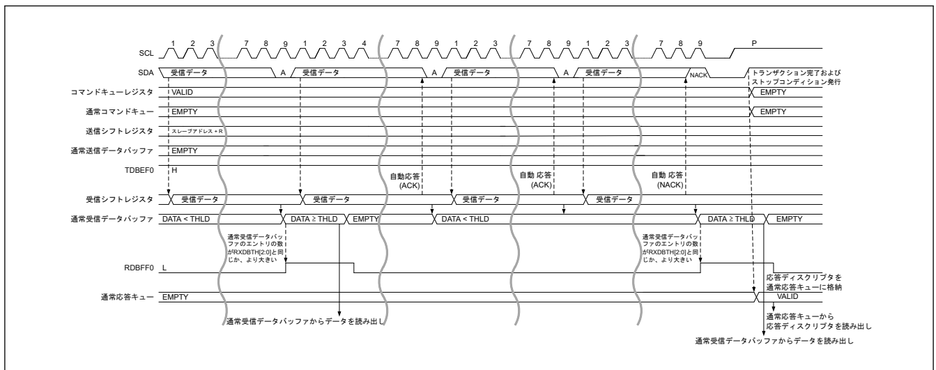
図 33.21 SDR データ読み出し転送タイミング (2/2)
