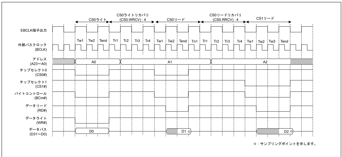
図 14.32 EBCLK 端子出力選択ビットで BCLK の 2 分周を選択した場合のリカバリサイクルの動作例（セパレートバスインタフェースによるノーマルアクセスの場合）（ m = 0 \sim 3 ）
