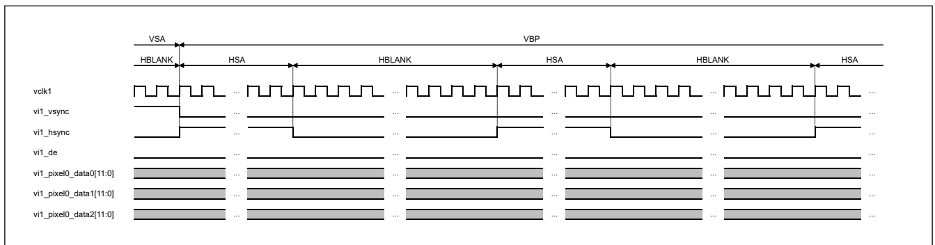
図 58.11 VSA 終了および VBP 開始
