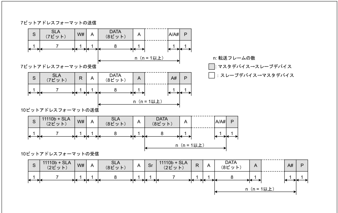
図 31.86 I 2 C バスフォーマット
