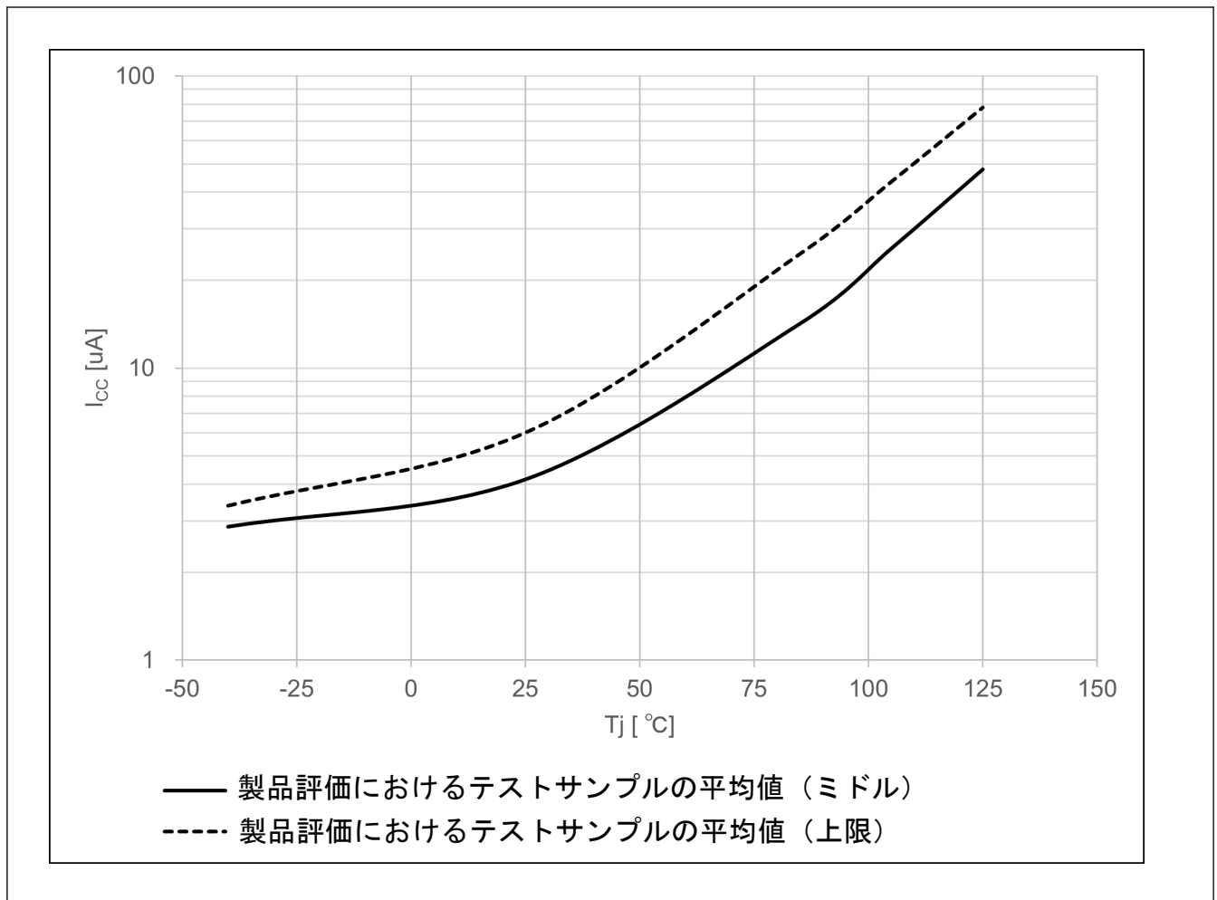
図 60.5 ディープソフトウェアスタンバイモード1における温度依存性 (参考データ)
