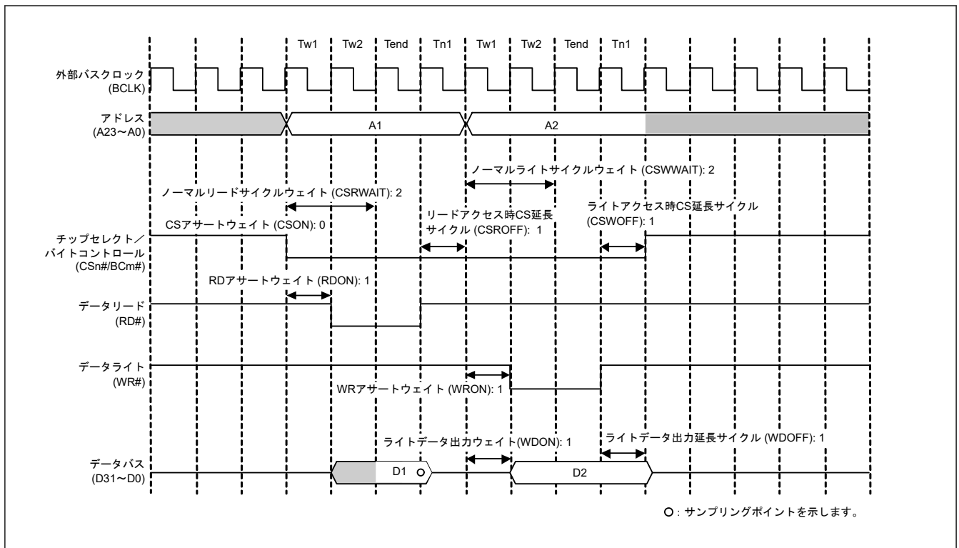
図 14.5 ノーマルアクセスの動作例（リード/ライト）(n = 0~7, m = 0~3)
