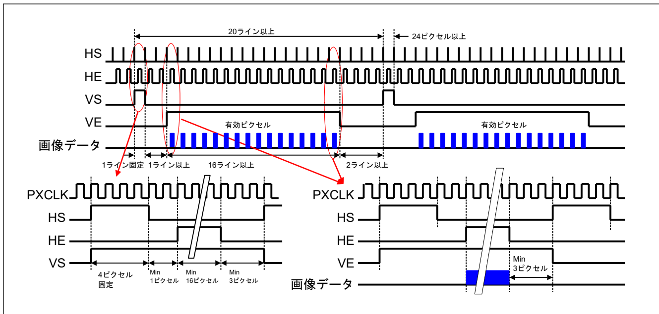
図 56.23 GLCDC 内の画像データキャリア信号
