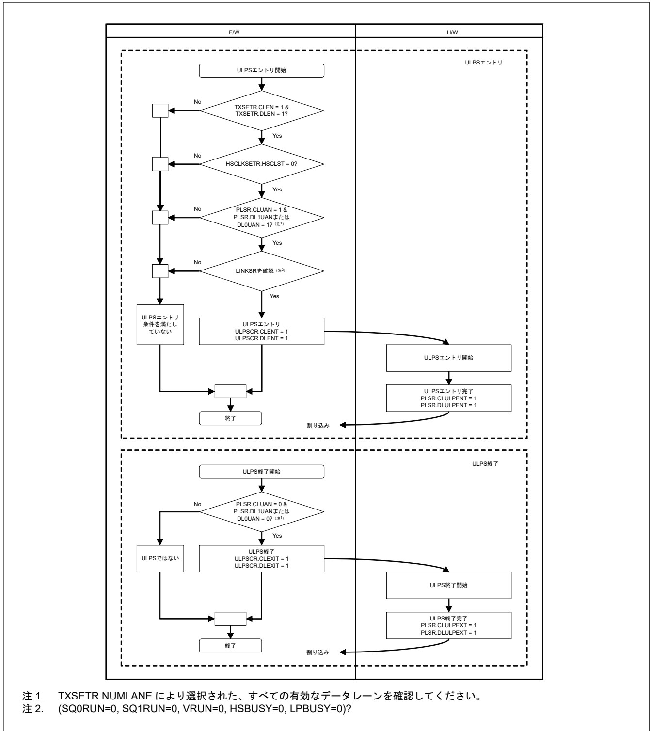
図 58.8 ULPS 遷移/復帰 (クロックレーンとデータレーン)
