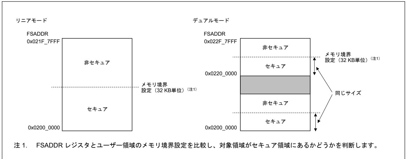
図 52.39 ユーザー領域内のセキュア領域と非セキュア領域 (セキュアエアリアスの場合)
