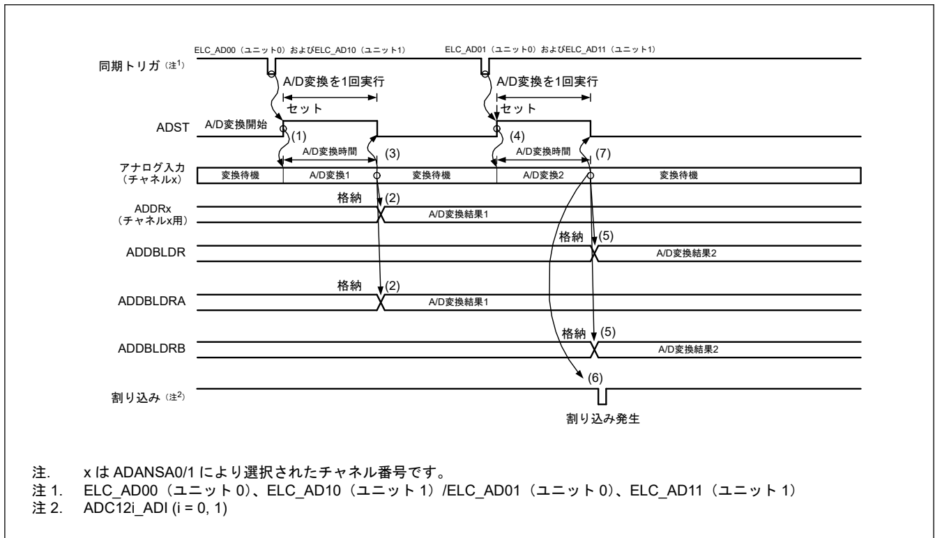
図 45.16 アナログ入力 (チャンネル x) と ELC_AD00 (ユニット 0)、ELC_AD10 (ユニット 1) /ELC_AD01 (ユニット 0)、ELC_AD11 (ユニット 1) の重複選択時のダブルトリガモード拡張動作例
