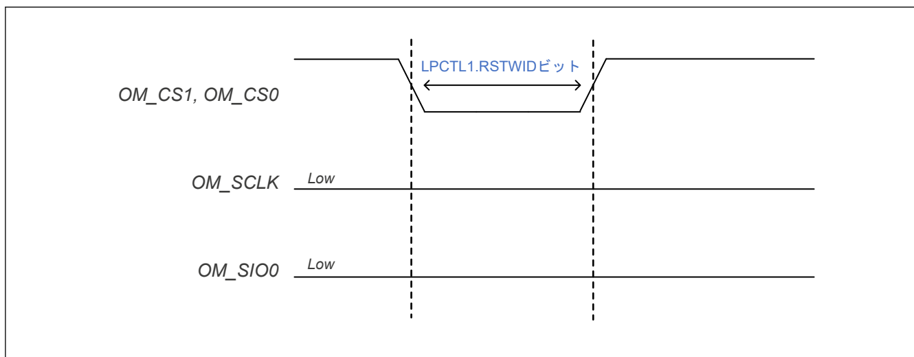
図 37.21 CS のみパターン
