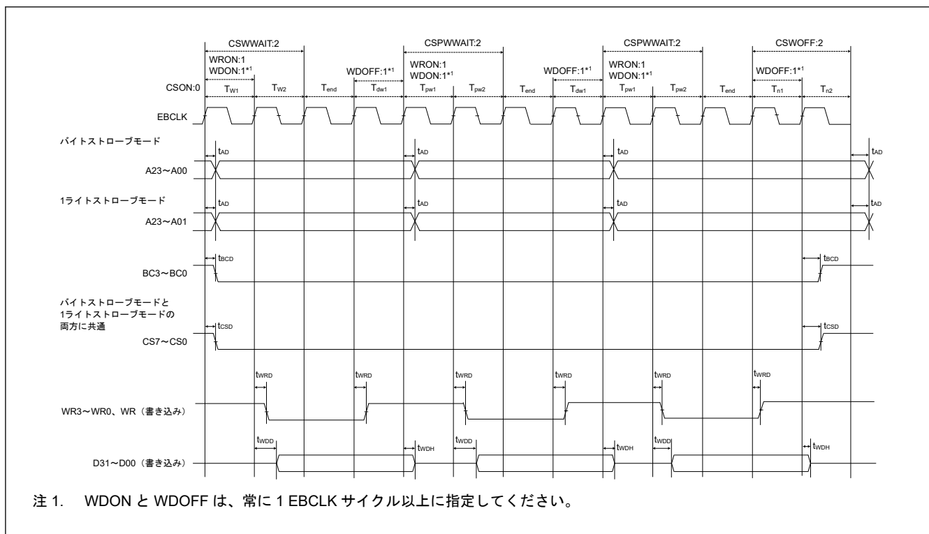
図 60.33 バスクロック同期を使用したページライトサイクルの外部バスタイミング
