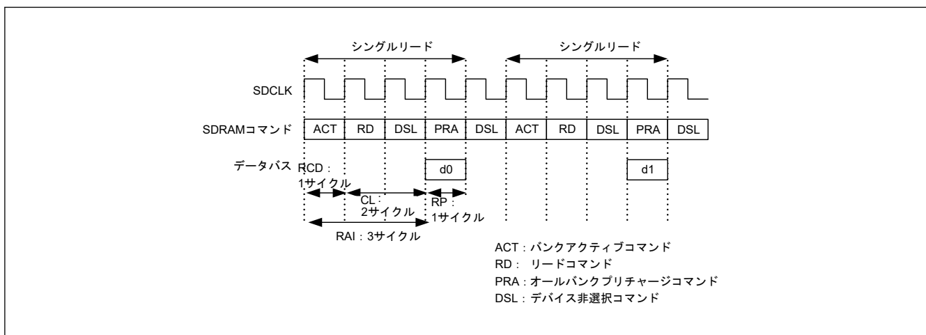
図 14.55 シングルリードタイミング例 (4)
