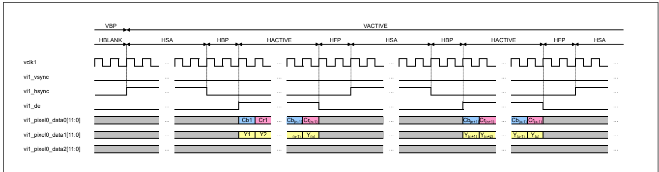
図 58.13 VBP 終了および VACTIVE 開始 (YCbCr 4: 2: 2)
