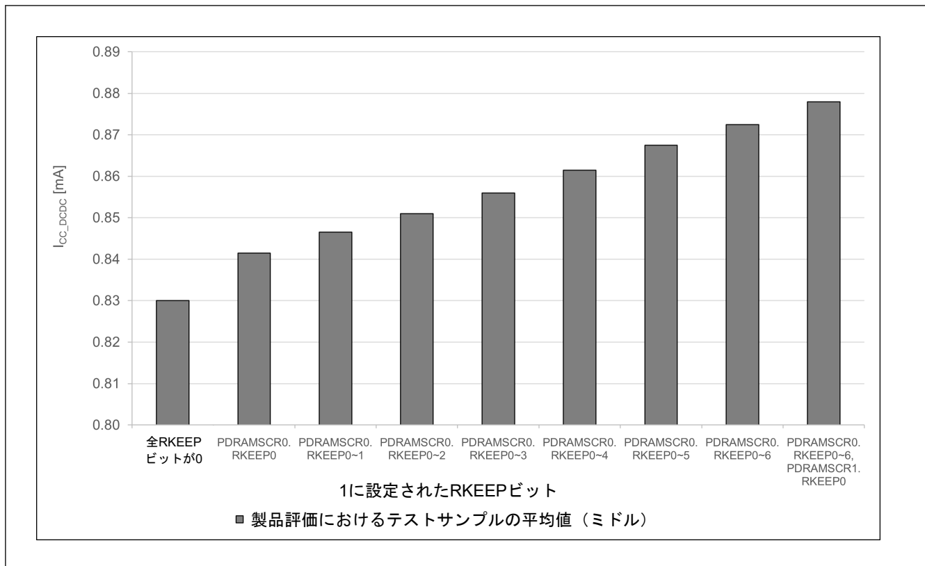
図 60.8 1 SRAM ステートあたりのソフトウェアスタンバイ電流 (参考データ)
