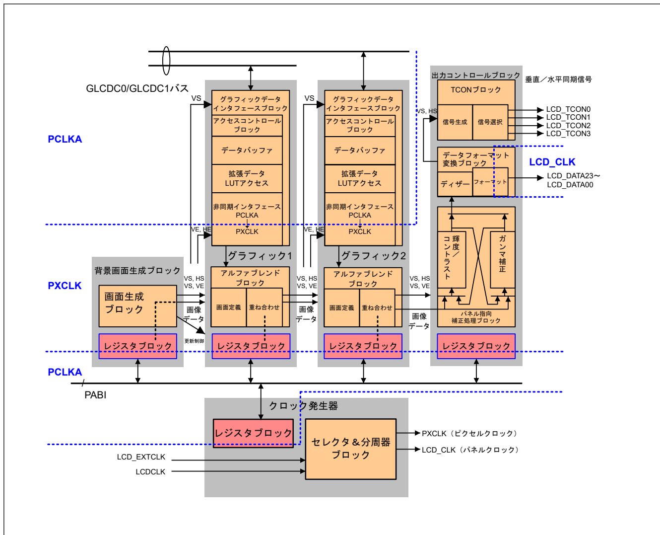
図 56.2 GLCDC の構成
