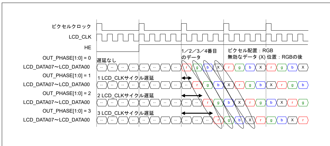
図 56.5 シリアル RGB888 (4 倍速) 出力タイミング
