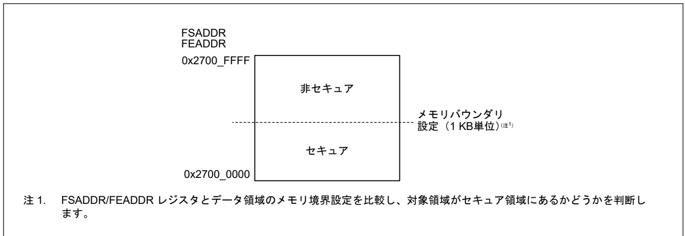
図 52.40 データ領域内のセキュア領域と非セキュア領域 (セキュアエアリアスの場合)
