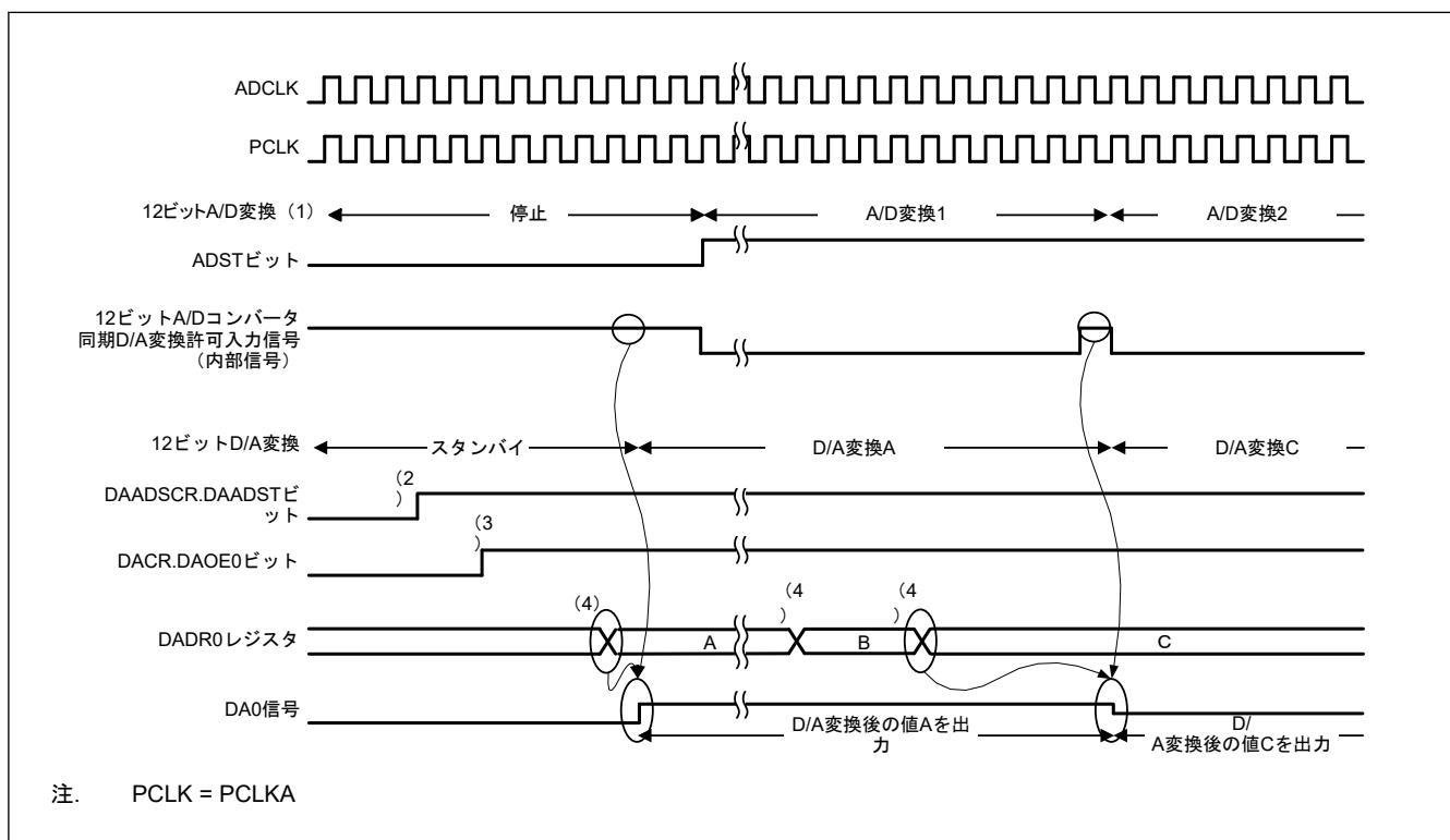
図 46.3 DAC12 を次に同期して変換する例：ADC12 (ユニット 1)
