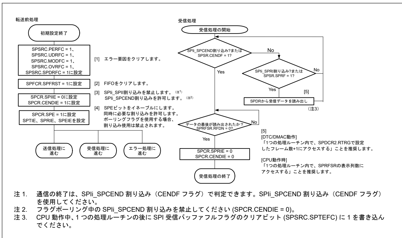
図 36.71 マスタモード時のソフトウェア処理フローチャート (受信のみ)
