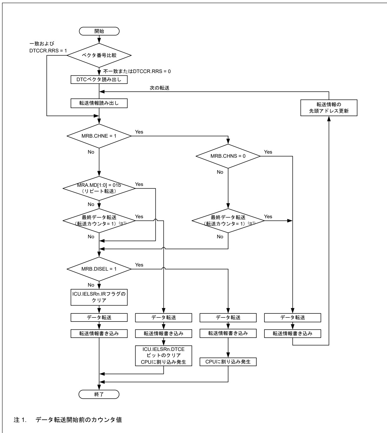
図 17.5 DTC 動作フローチャート
