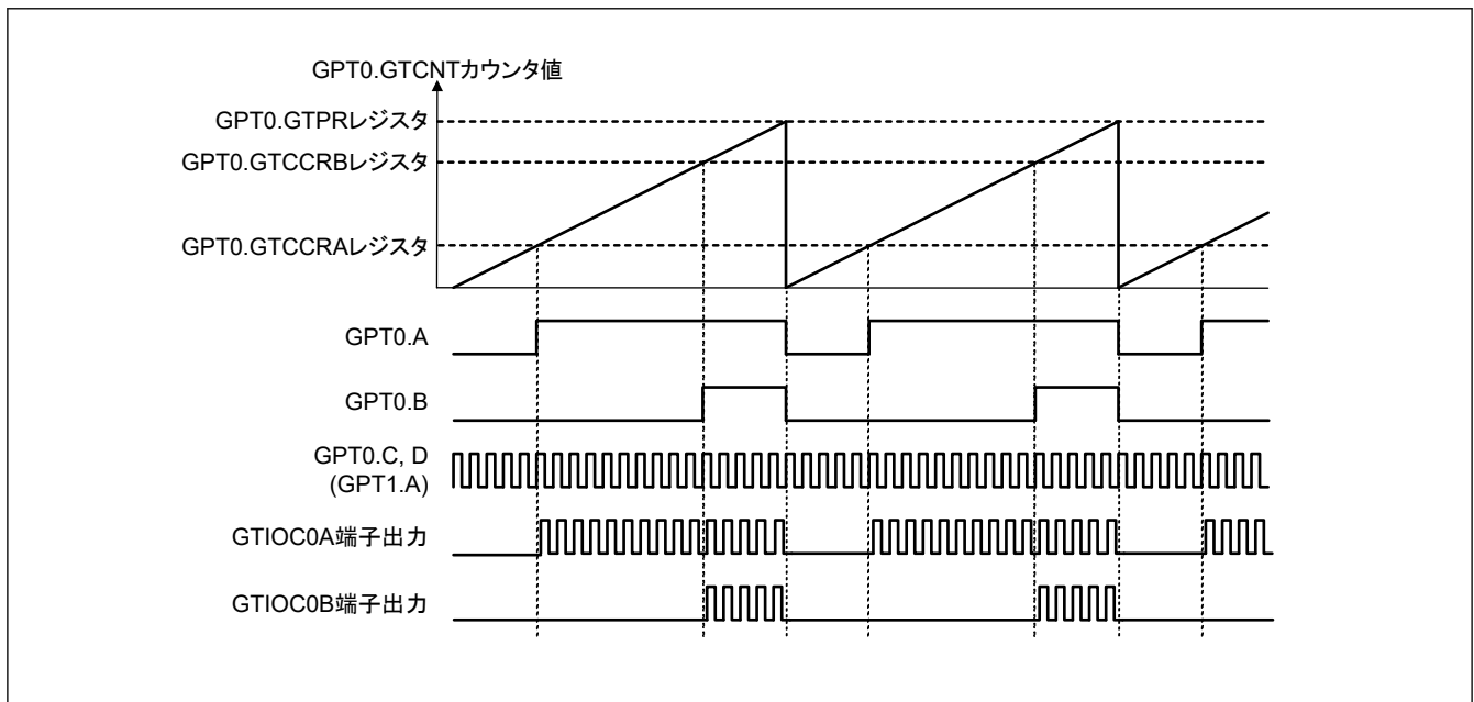
図 21.69 チャンネル間論理演算の例
