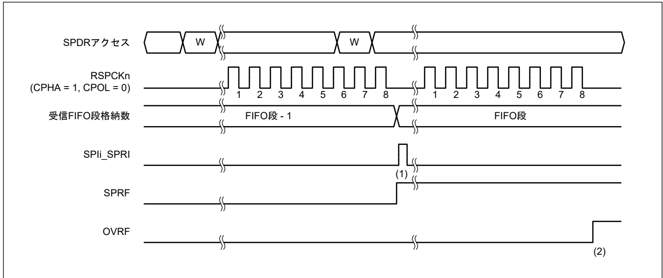
図 36.30 SPCR.TXMD[1:0] = 00b の場合の動作例
