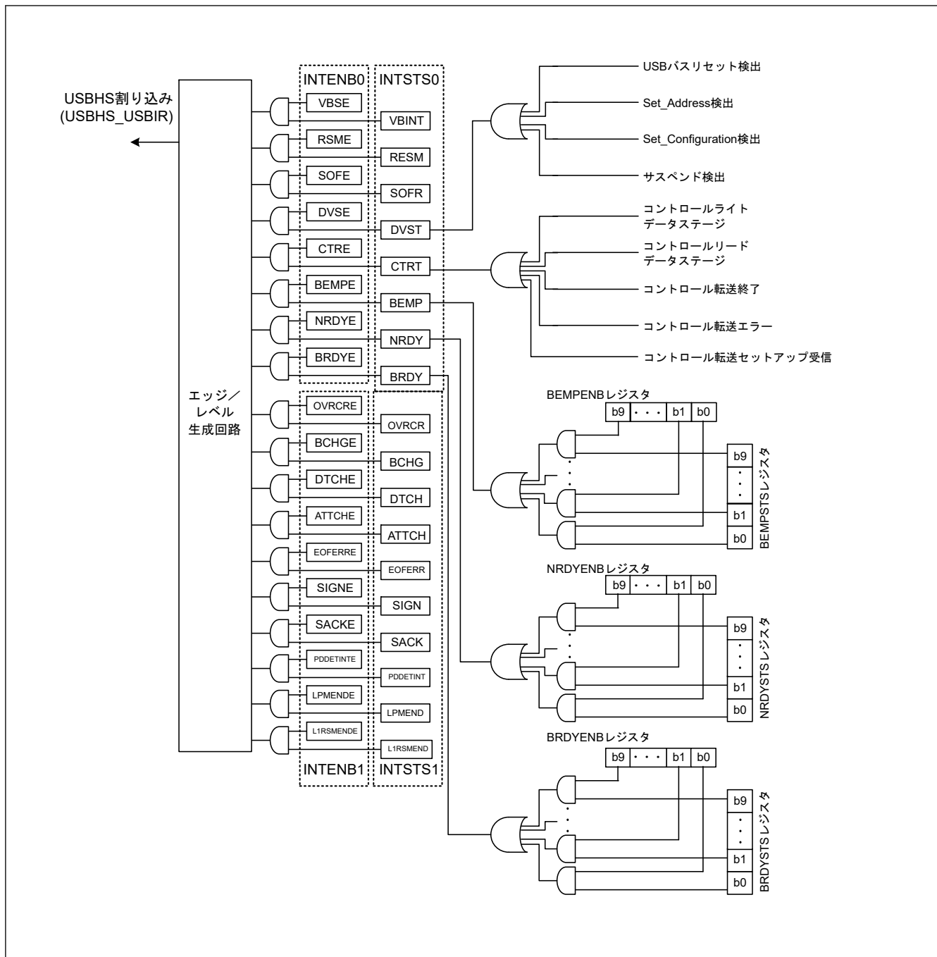
図 30.4 USBHS 割り込み関連回路
