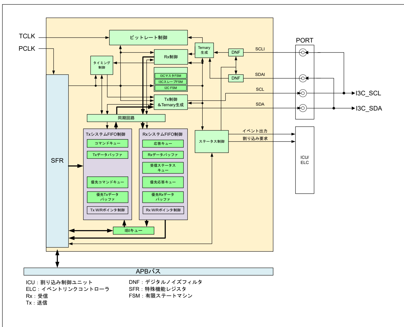
図 33.1 I3C ブロック図
