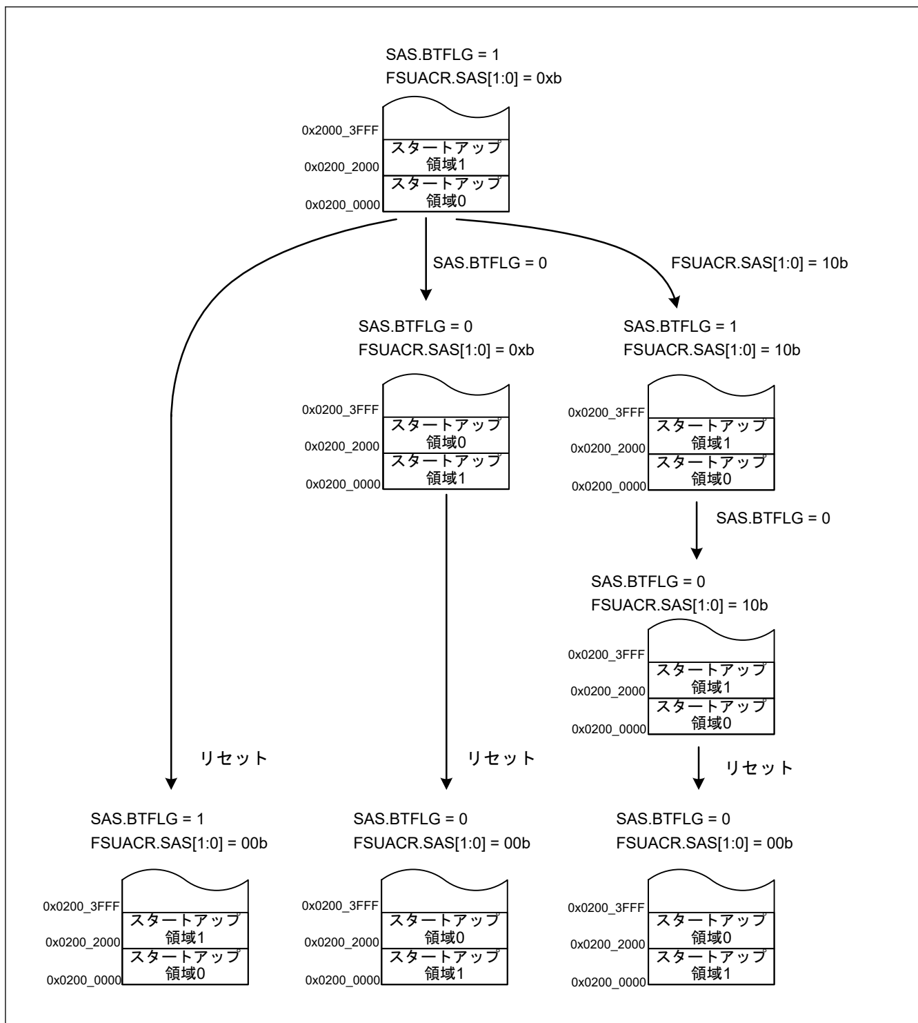
図 52.30 スタートアッププログラム保護設定の遷移例 1 (セキュアエリアの場合)
