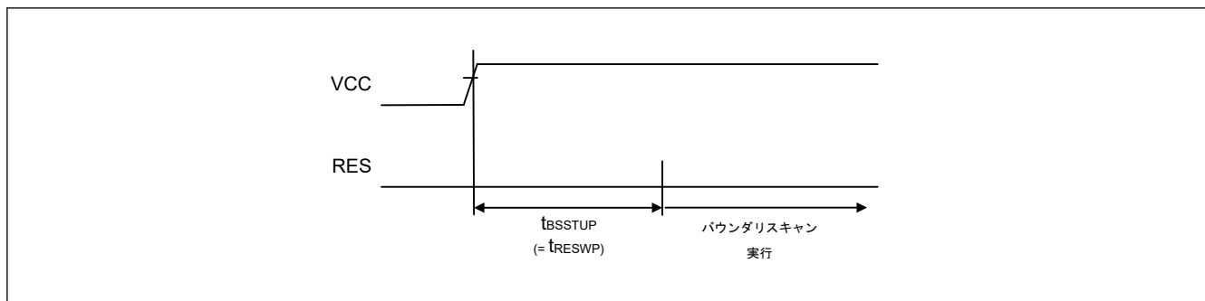
図 52.89 バウンダリスキャン回路起動タイミング
