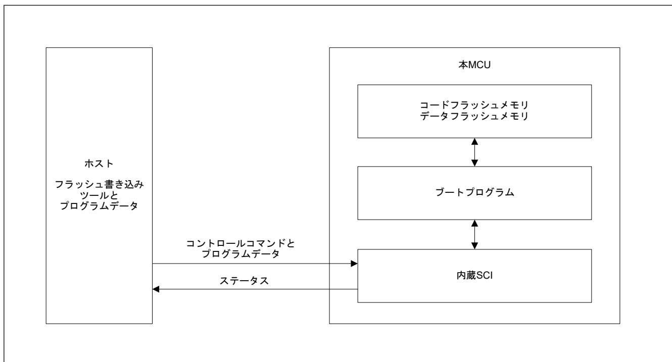
図 49.47 ブートモード（SCI インタフェース）時のシステム構成
