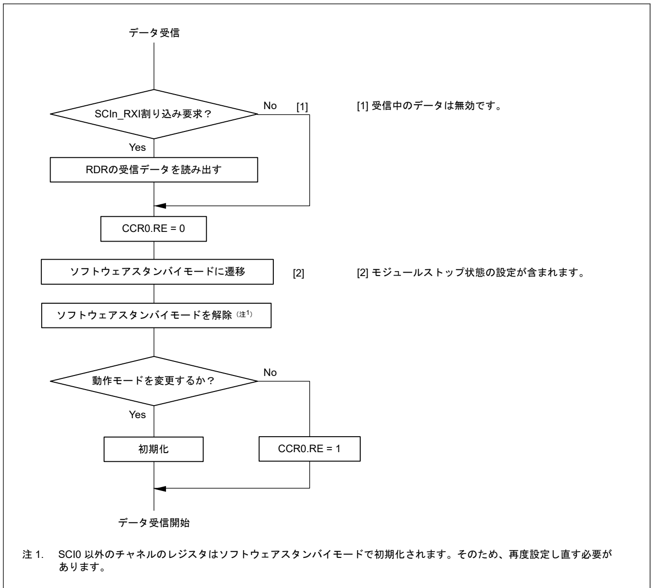
図 30.120 受信時にソフトウェアスタンバイモードへ移行する場合のフローチャート例
