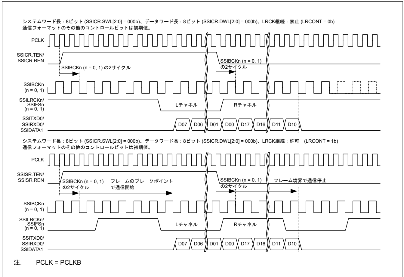
図 37.33 LR クロック/フレーム同期継続の動作例
