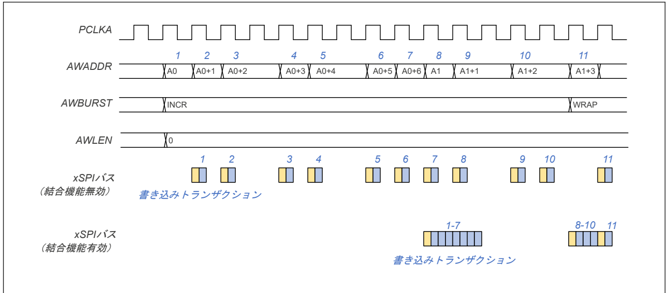
図 35.14 結合機能
