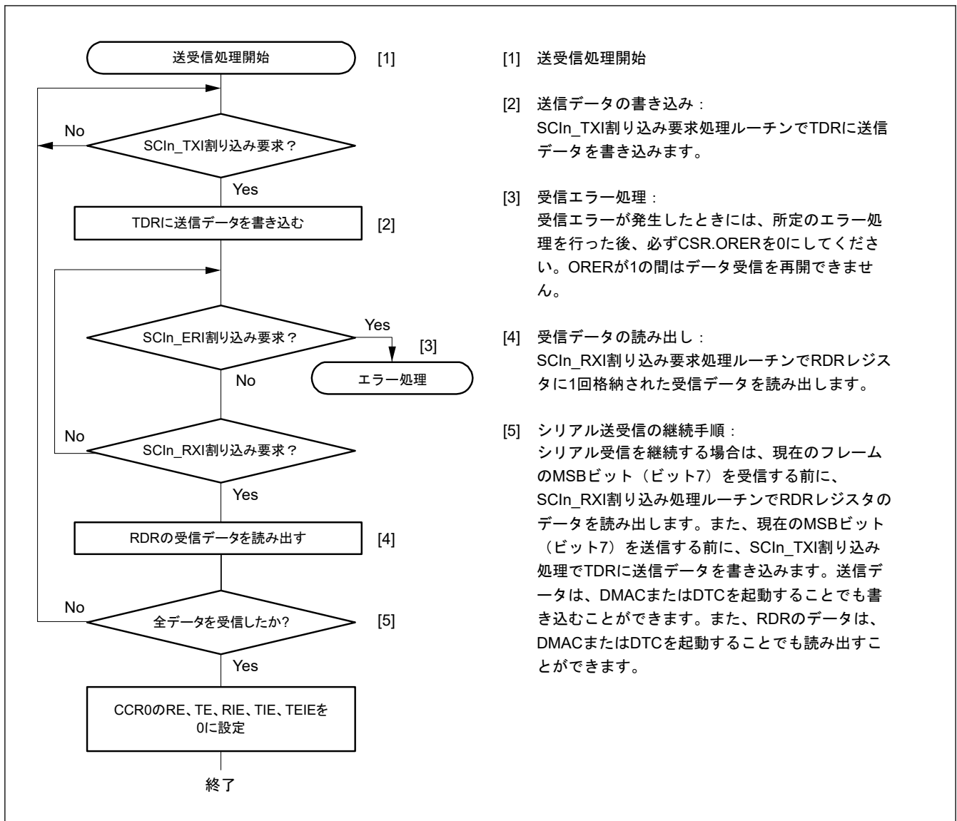
図 30.71 クロック同期式モードにおけるシリアル同時送受信動作のフローチャート例（非 FIFO 選択時）
