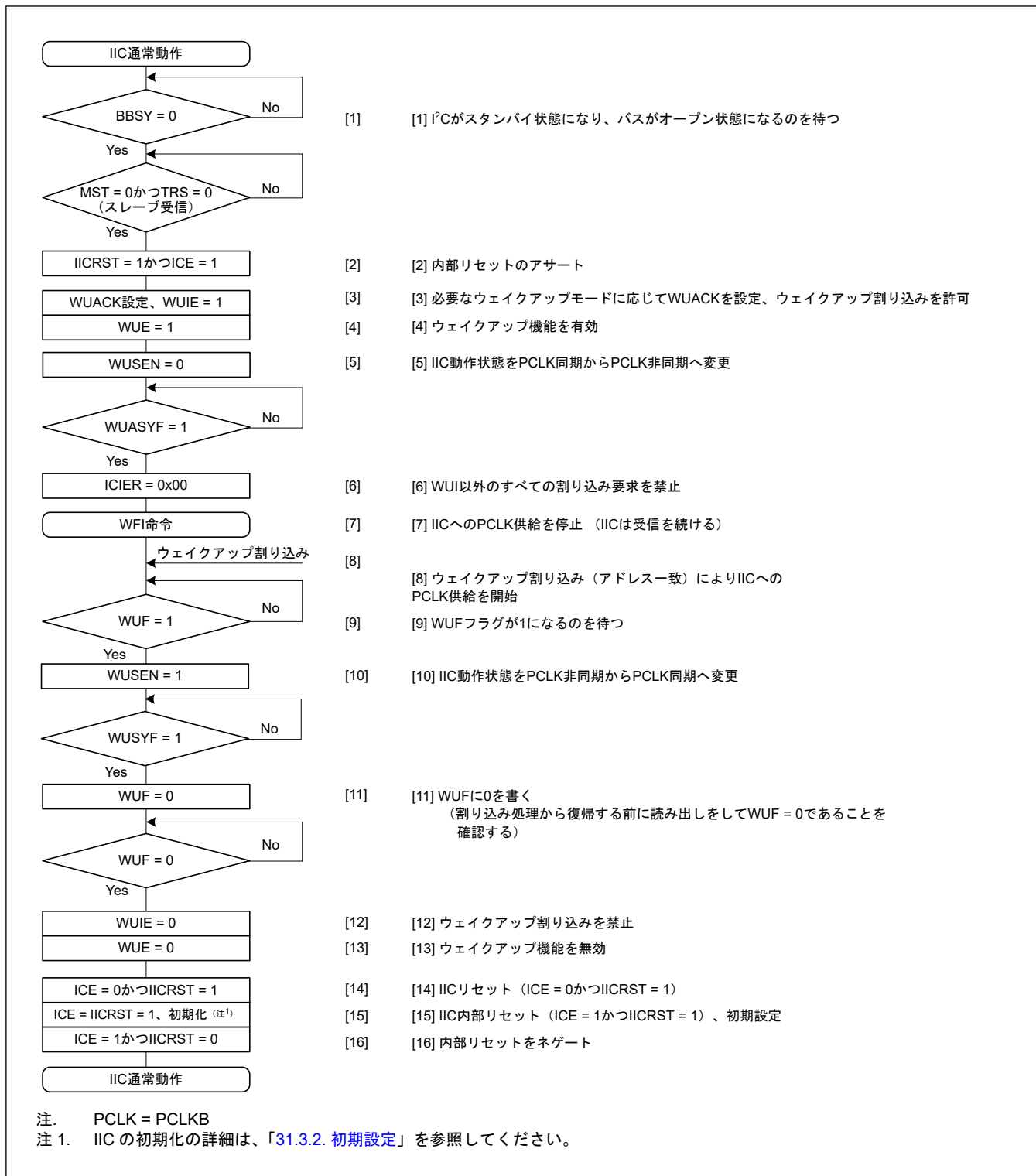
図 31.35 コマンドリカバリモードとEEP 応答モードの動作例 (スレーブアドレス一致時のウェイクアップ割り込みによるウェイクアップの場合)
