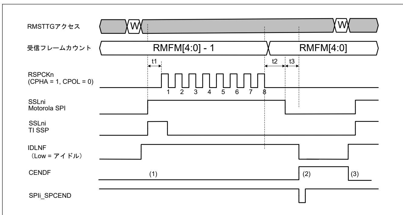
図 34.39 RMFM[4:0] ≠ 0 時の通信終了割り込み動作例 (受信専用マスタモード/Motorola-SPI)
