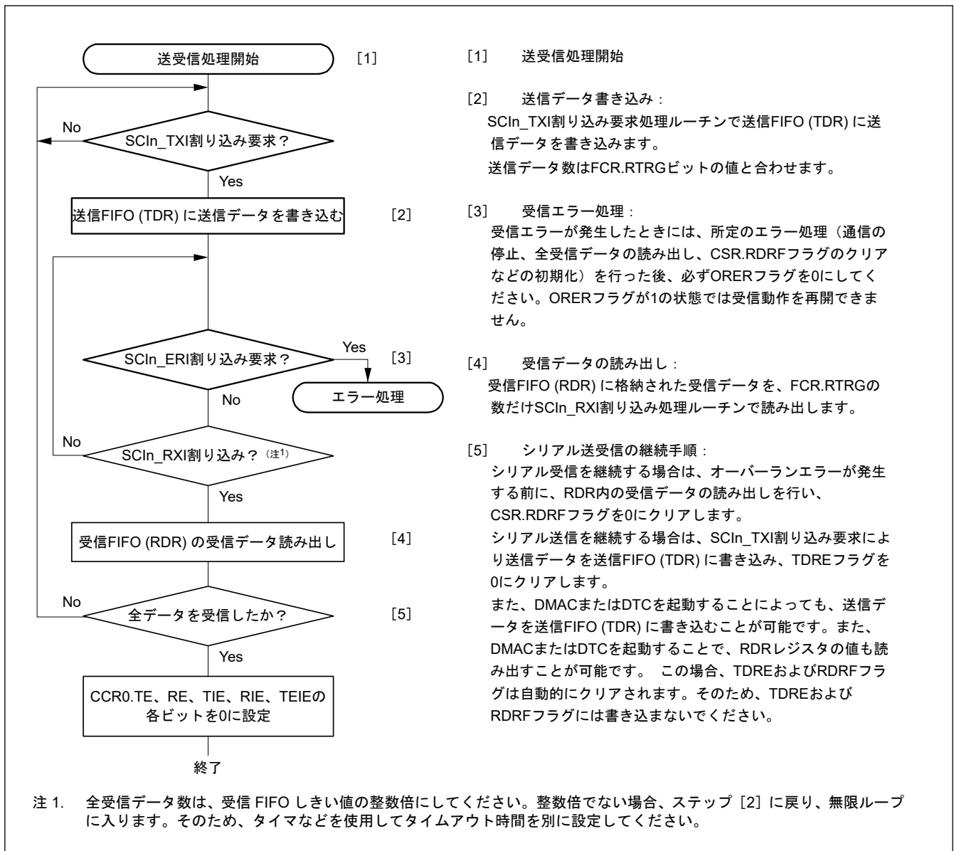
図 30.72 クロック同期式モードにおけるシリアル同時送受信動作のフローチャート例 (FIFO 選択時)
