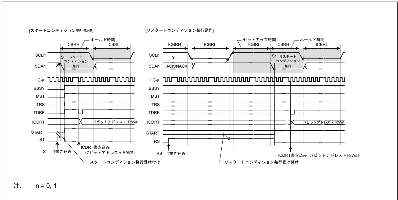
図 31.45 スタートコンディション/リスタートコンディション発行動作タイミング (ST、RS ビット)
