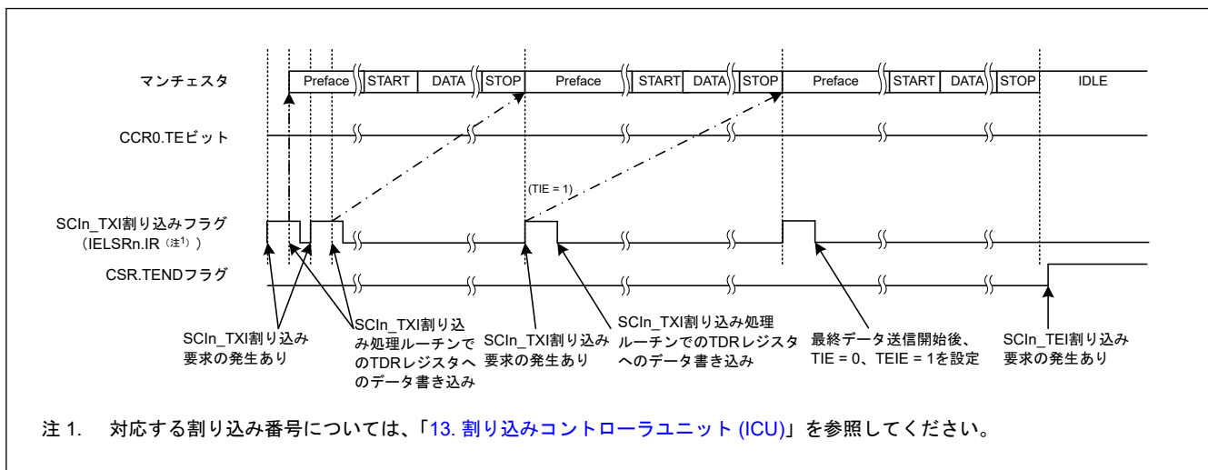
図 30.54 マンチェスタモードにおけるシリアル送信の終了動作の例 (プレフィスあり、CTS 機能なし)
