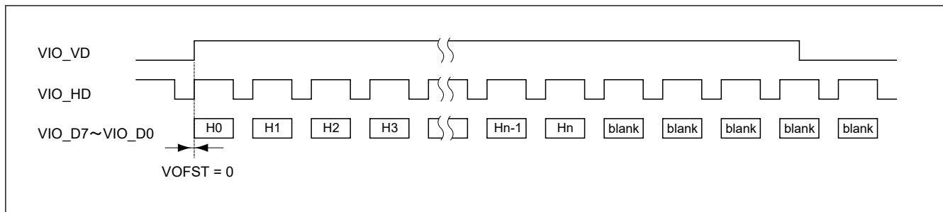
図 50.18 VD がデータイネーブル信号の場合のタイミング
