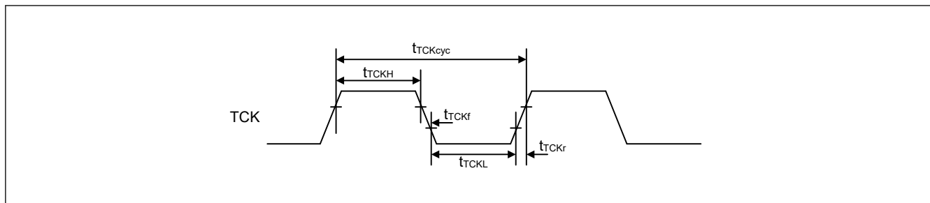
図 52.86 バウンダリスキャン TCK タイミング
