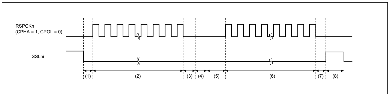
図 34.57 SSLKP ビット (BFDS = 0, SPFRF = 0) を使用したバースト転送の動作例
