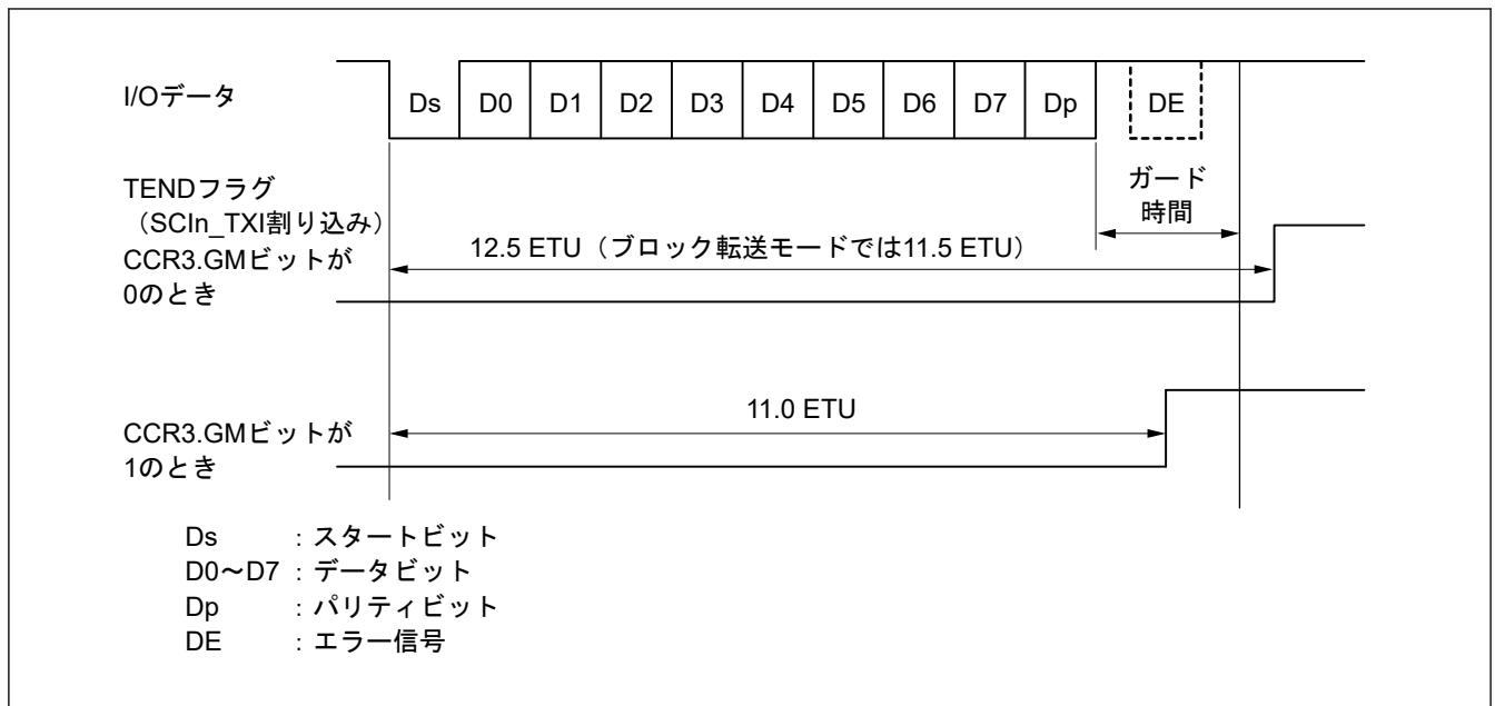
図 30.81 送信中の CSR.TEND フラグの発生タイミング
