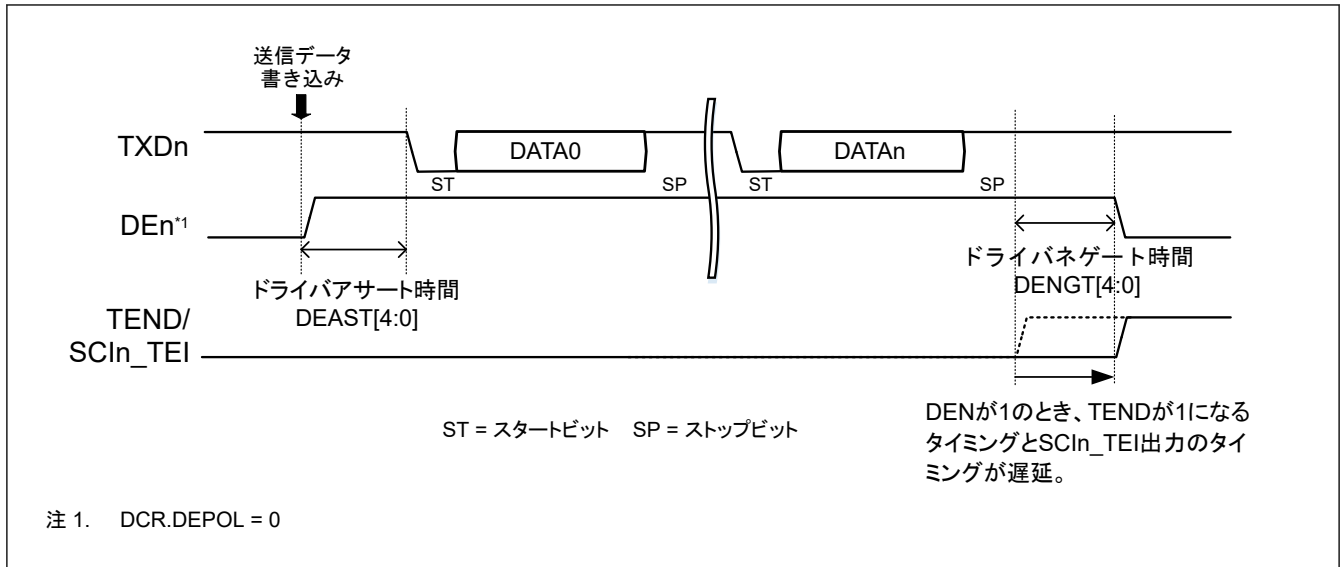
図 30.114 RS-485 ドライバコントロールの DE 信号出力のイメージ波形
