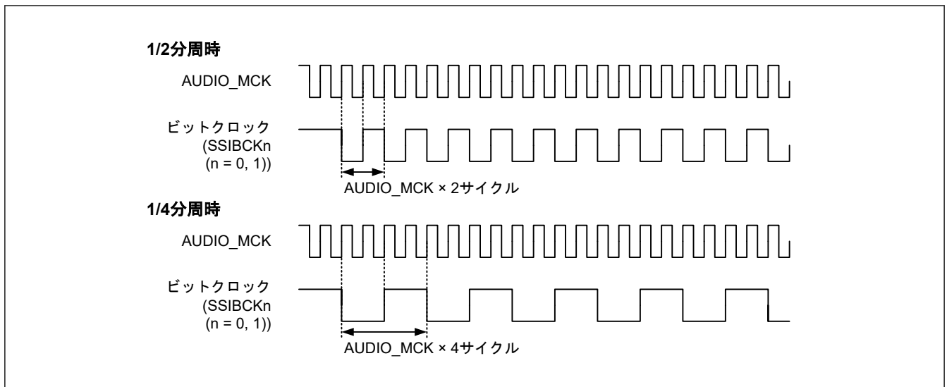
図 37.6 マスタモード通信時のサンプリング周波数
