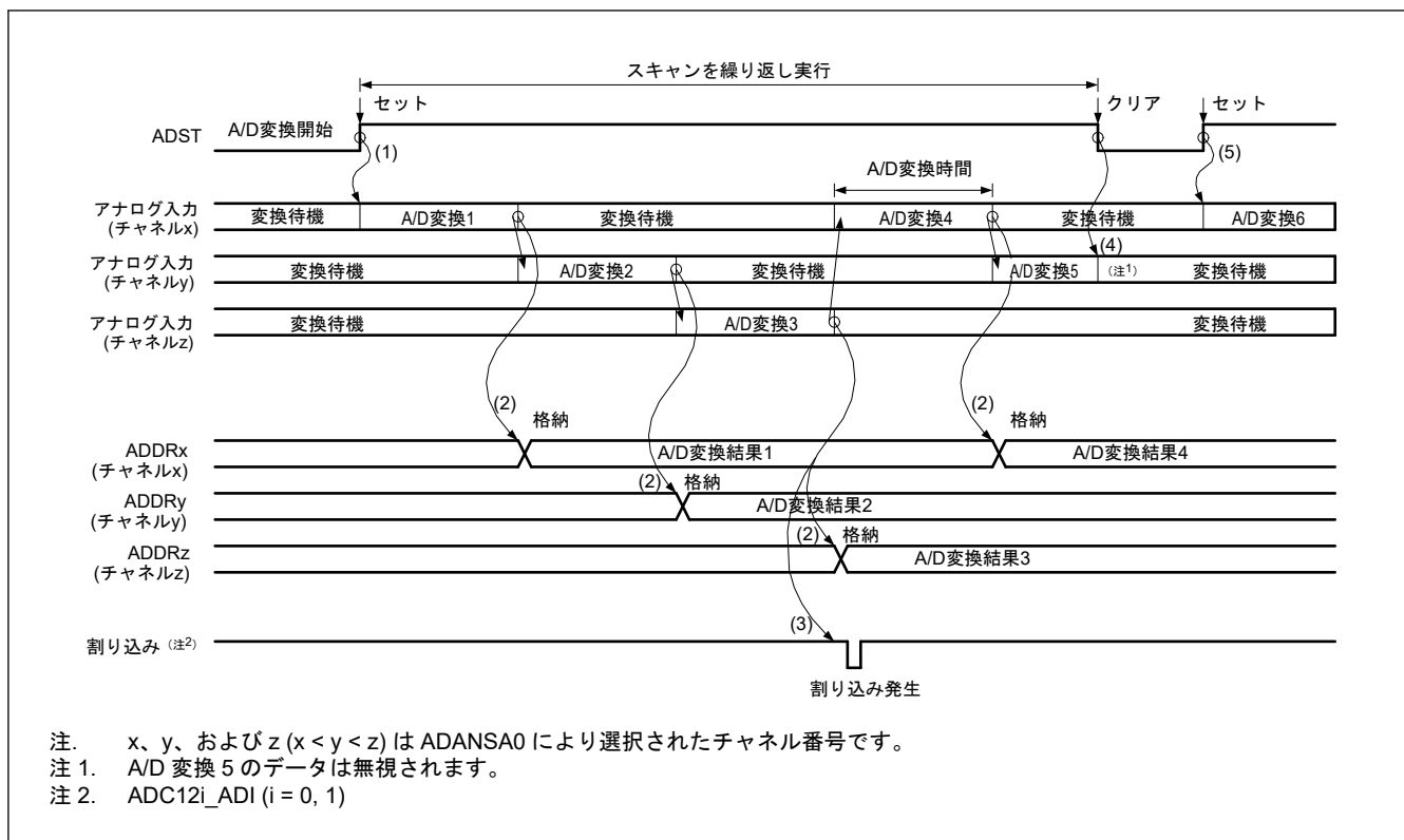
図 42.17 連続スキャンモードの基本動作例 (アナログ入力 (チャンネル x~z) 選択)
