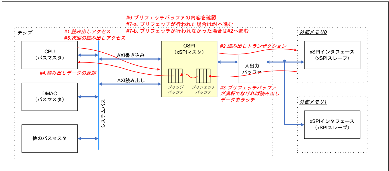
図 35.18 プリフェッチ許可時のメモリ領域の読み出しアクセス
