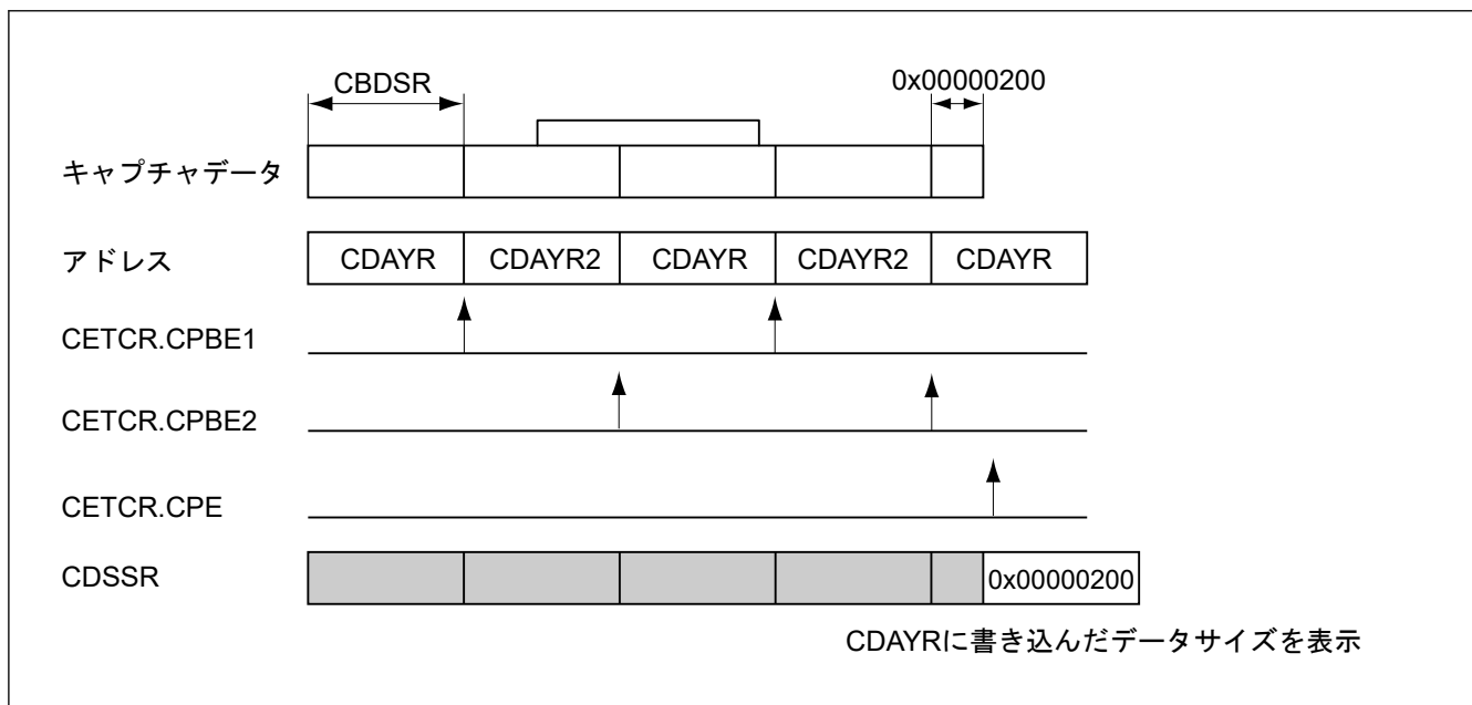
図 50.49 バンドル書き込み時の CDSSR 動作タイミングイメージ図 (バンドル書き込み終了とキャプチャ終了が異なる場合)
