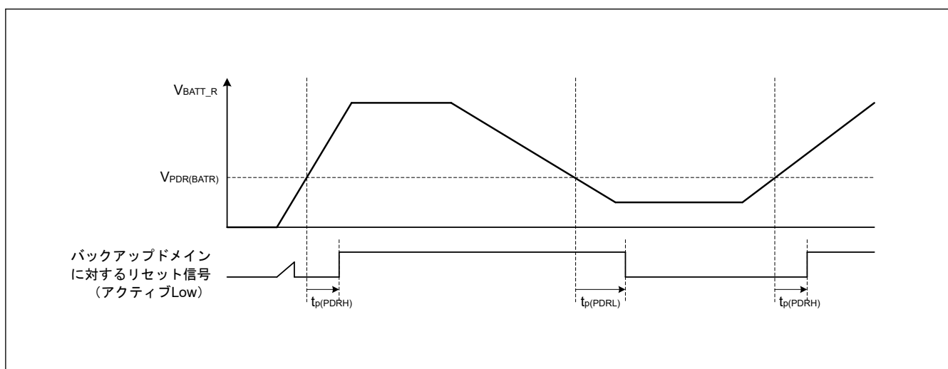
図 52.84 バックアップドメインリセット特性
