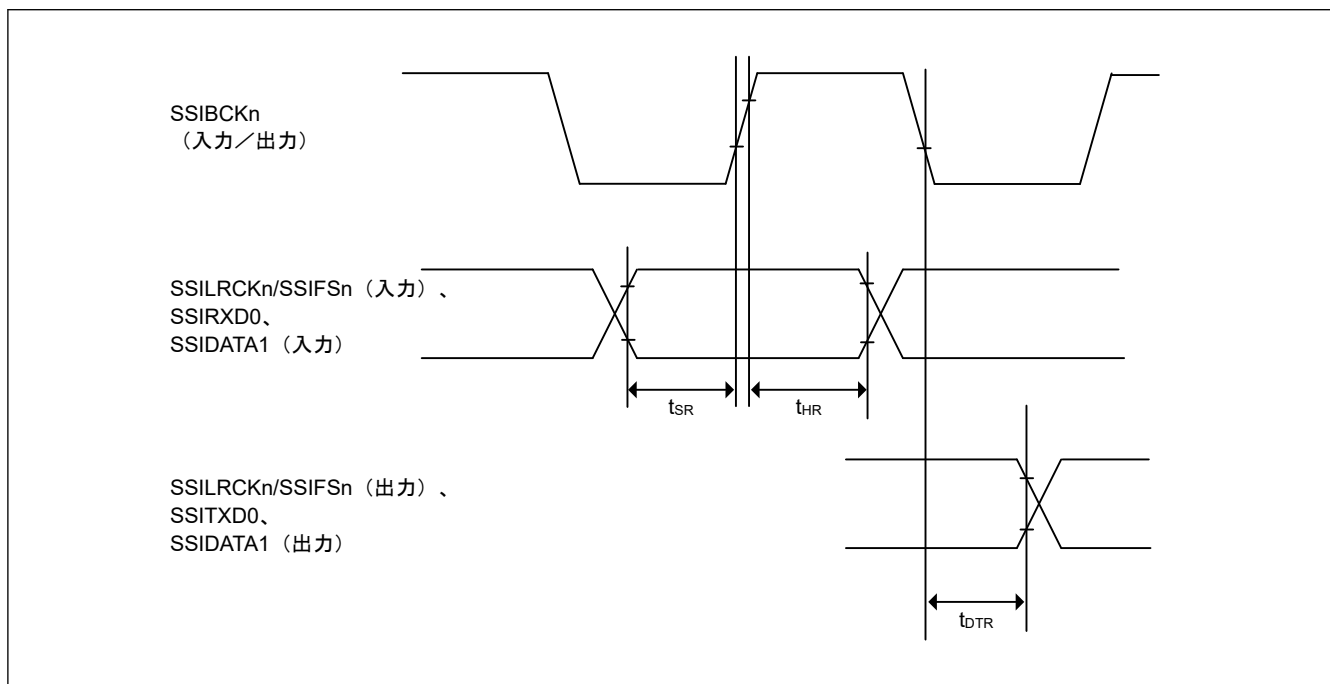
図 52.58 SSICR.BCKP = 0 の場合の SSIE データ送受信タイミング
