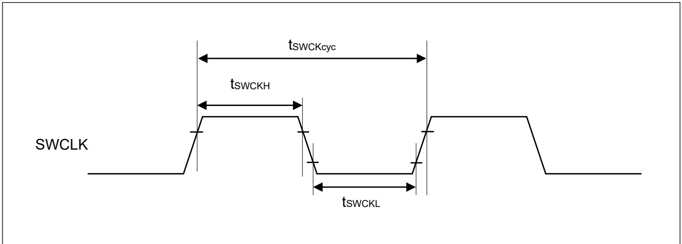
図 52.92 SWD SWCLK タイミング
