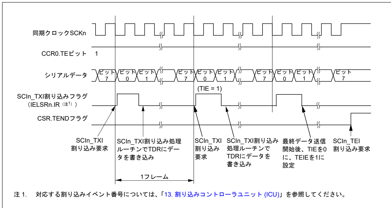
図 30.64 クロック同期式モードにおけるシリアル送信の動作例 (送信中～送信終了時)
