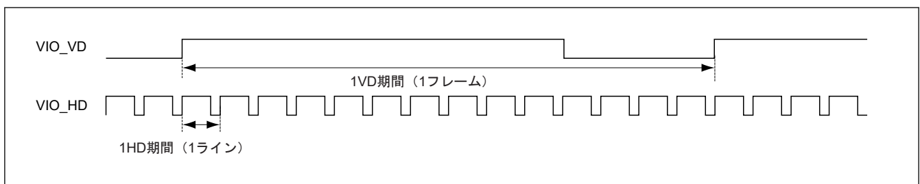
図 50.3 フレームタイミング
