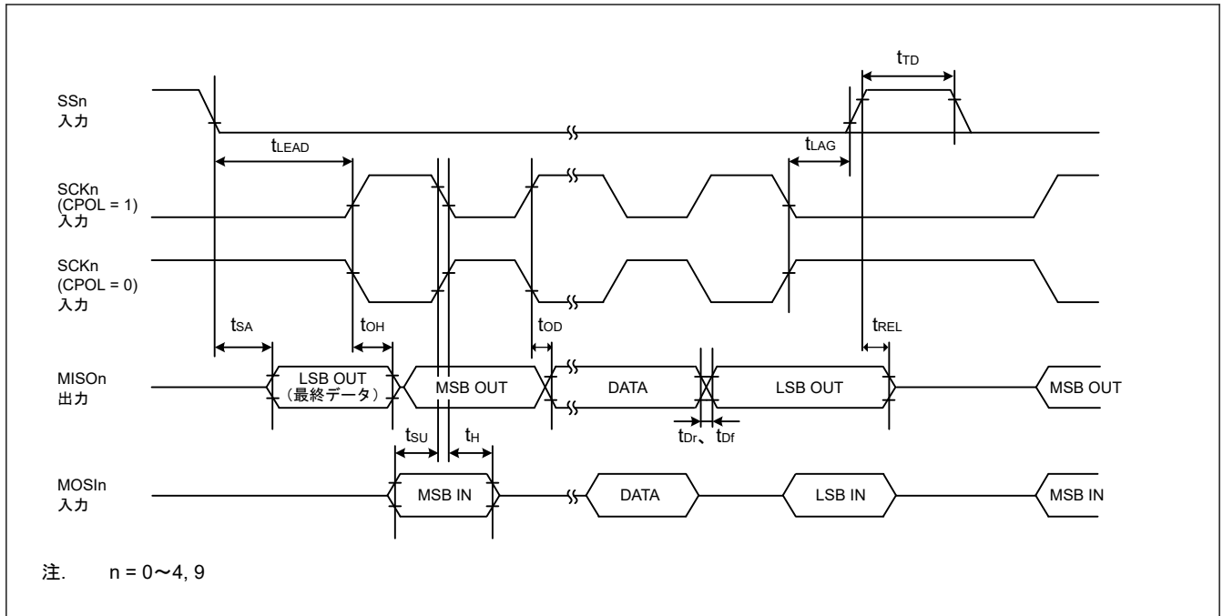
図 52.40 SCI 簡易 SPI モードタイミング (スレープ、CPHA = 1)
