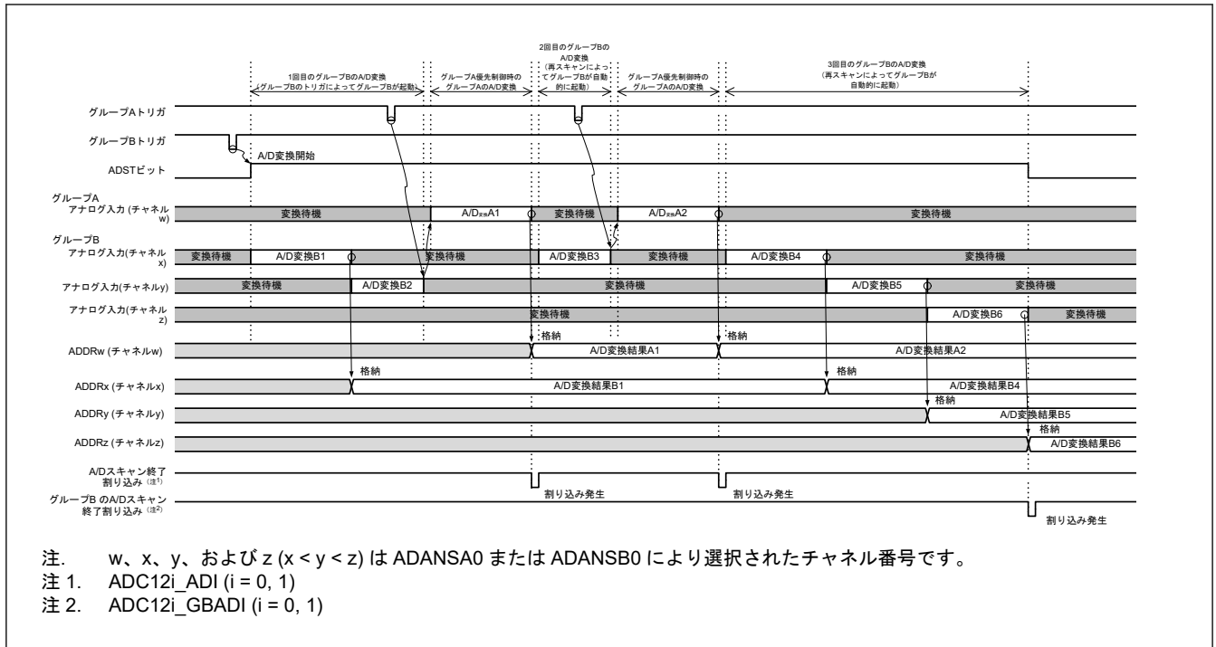
図 42.28 グループ優先動作の例 1-2 : グループ B 再スキャン中のグループ A トリガ入力、再スキャンあり (ADGSPCR.GBRSCN = 1、ADGSPCR.GBRP = 0、および ADGSPCR.LGRRS = 0 の場合)
