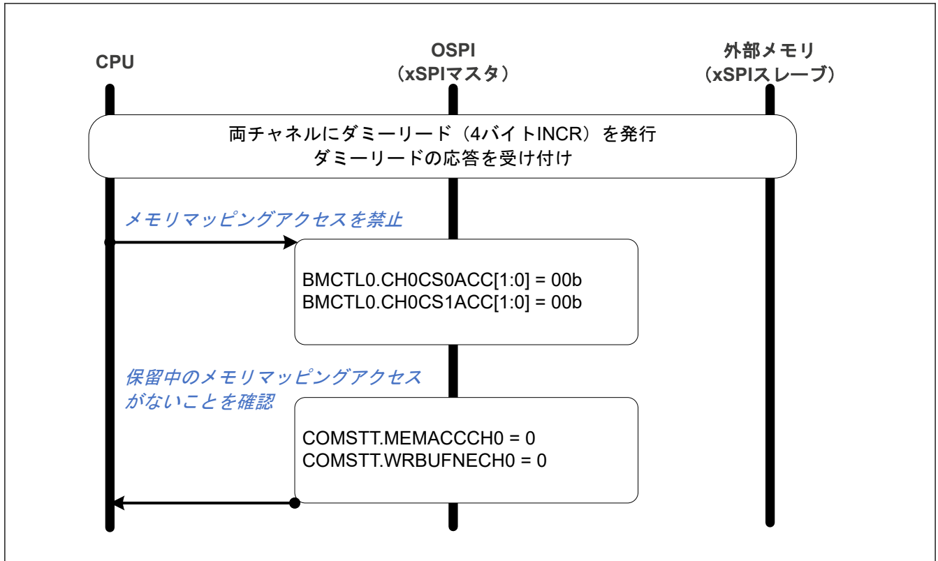
図 35.28 メモリマッピング停止のフロー
