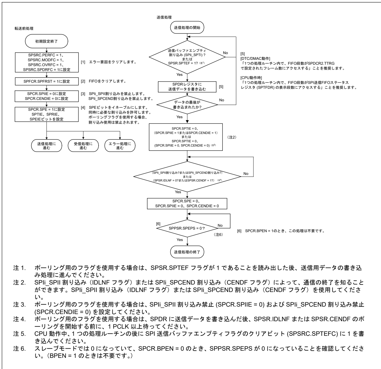
図 34.64 マスタモードでの送信フロー
