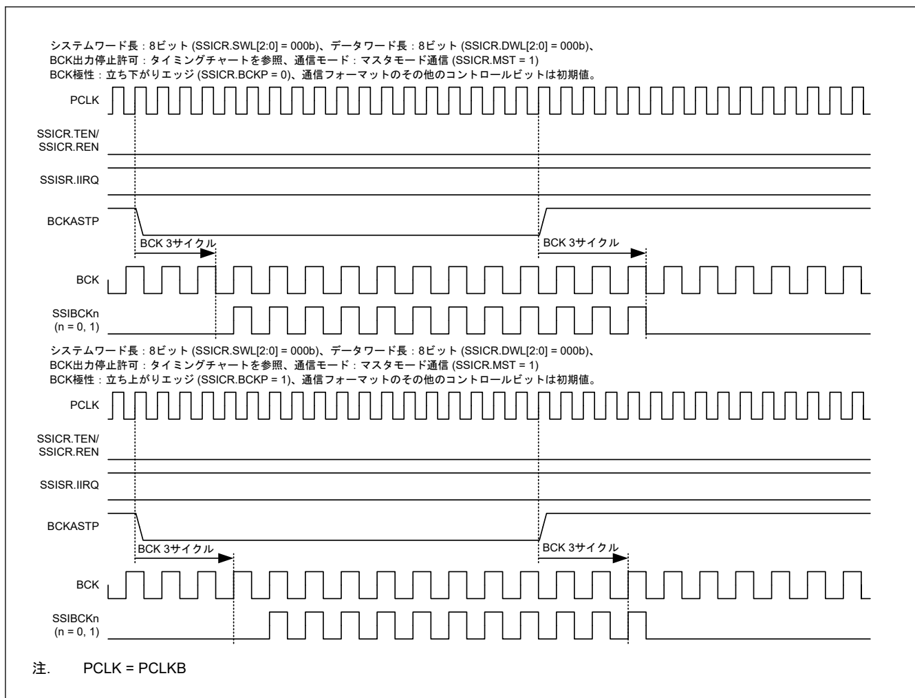
図 37.34 BCKASTP ビットの動作例 (アイドル状態の場合)
