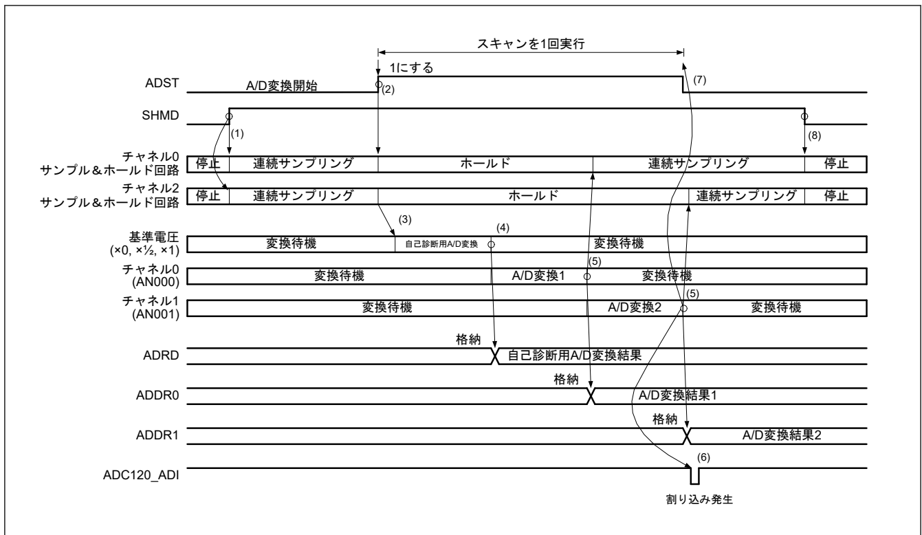
図 42.13 シングルスキャンモードの動作例 (チャンネル専用サンプル&ホールド回路使用、自己診断で AN000 および AN001 選択、連続サンプリング有効)
