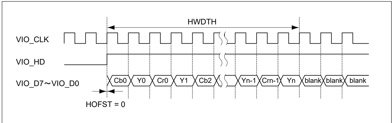
図 50.22 水平キャプチャタイミング
