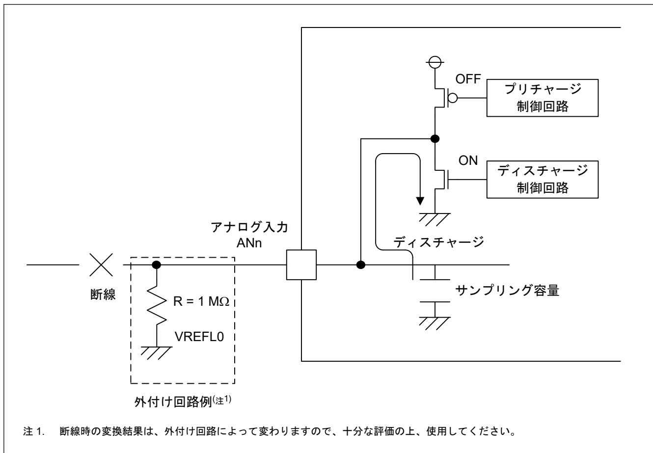
図 42.40 ディスチャージを選択した場合の断線検出例
