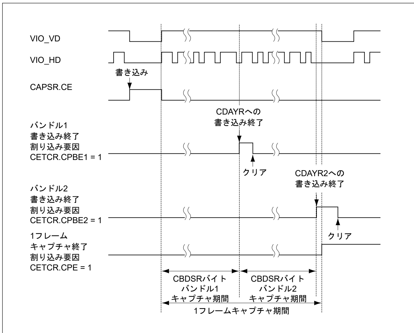
図 50.43 書き込み終了割り込みのタイミング (データイネーブル取り込み時)
