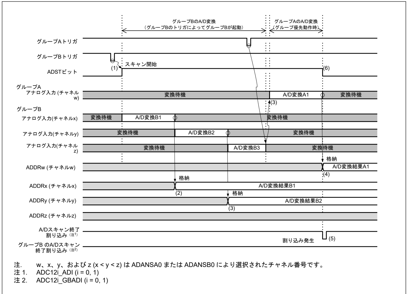
図 42.30 グループ優先動作の例 1-4 : グループ B スキャン中のグループ A トリガ入力、再スキャンなし (ADGSPCR.GBRSCN = 0, ADGSPCR.GBRP = 0, および ADGSPCR.LGRRS = 0 の場合)
