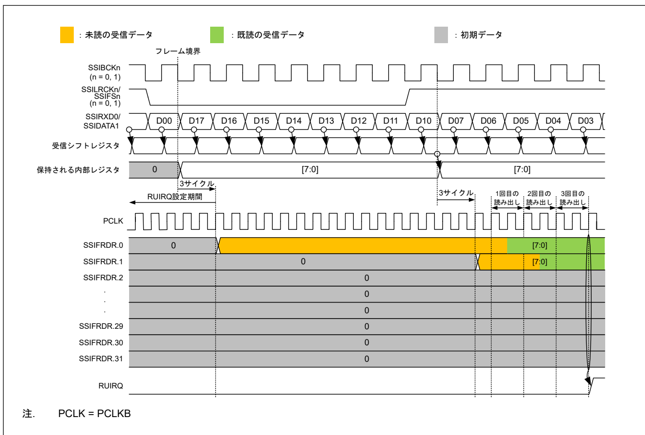
図 37.17 RUIRQ 設定タイミング
