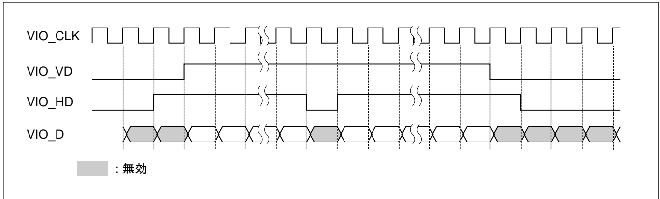
図 50.13 データイネーブル取り込みタイミング (VD が High の期間外に HD がアサート (High))
