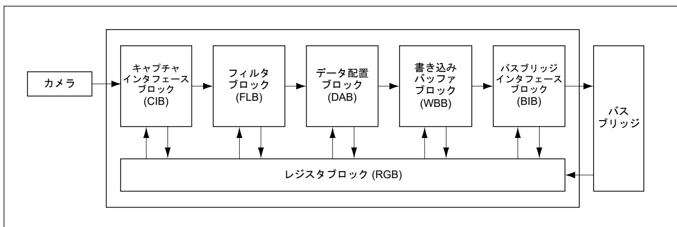
図 50.1 CEU のブロック図
