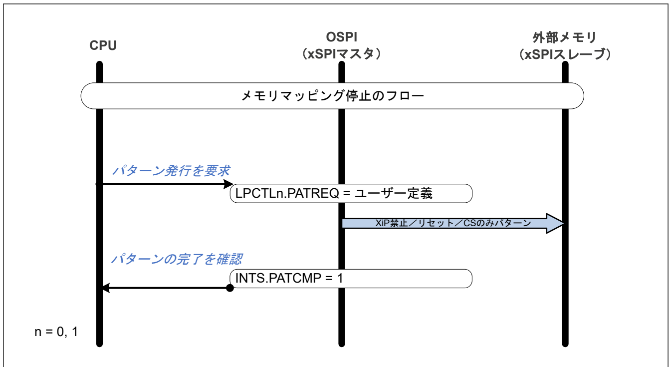
図 35.29 パターン要求のフロー
