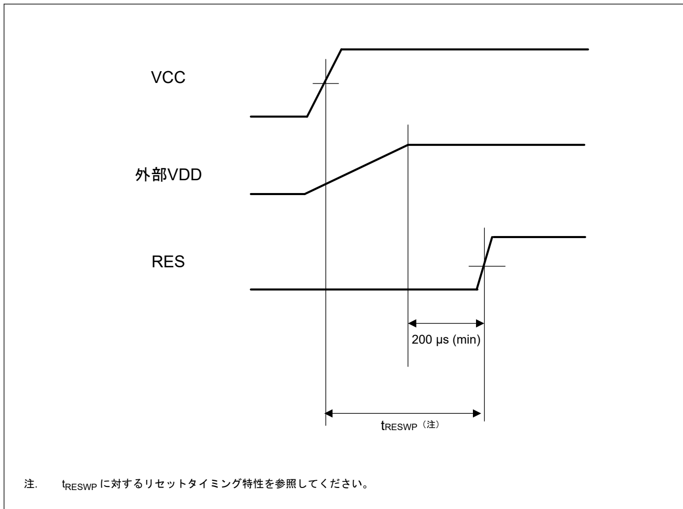
図 51.4 外部 VDD モードの電源起動シーケンス (RES 端子を使用する場合)
