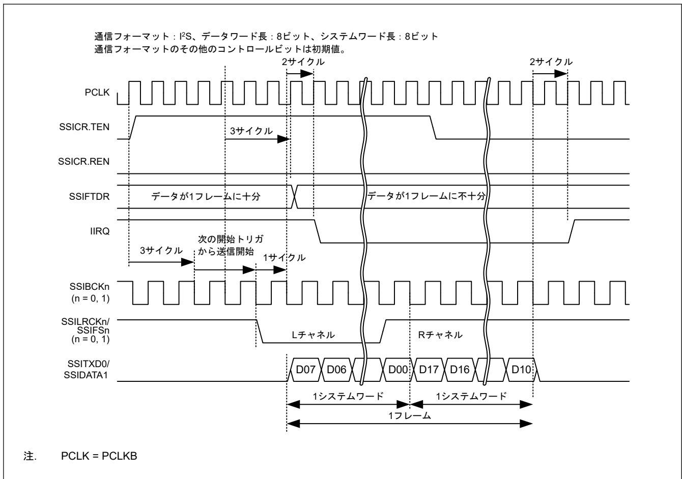
図 37.14 IIRQ 設定タイミング (送信)
