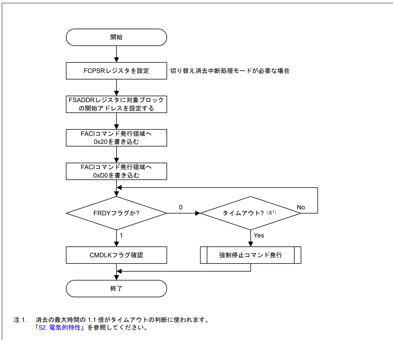
図 49.15 ブロックイレースコマンドの使用フロー
