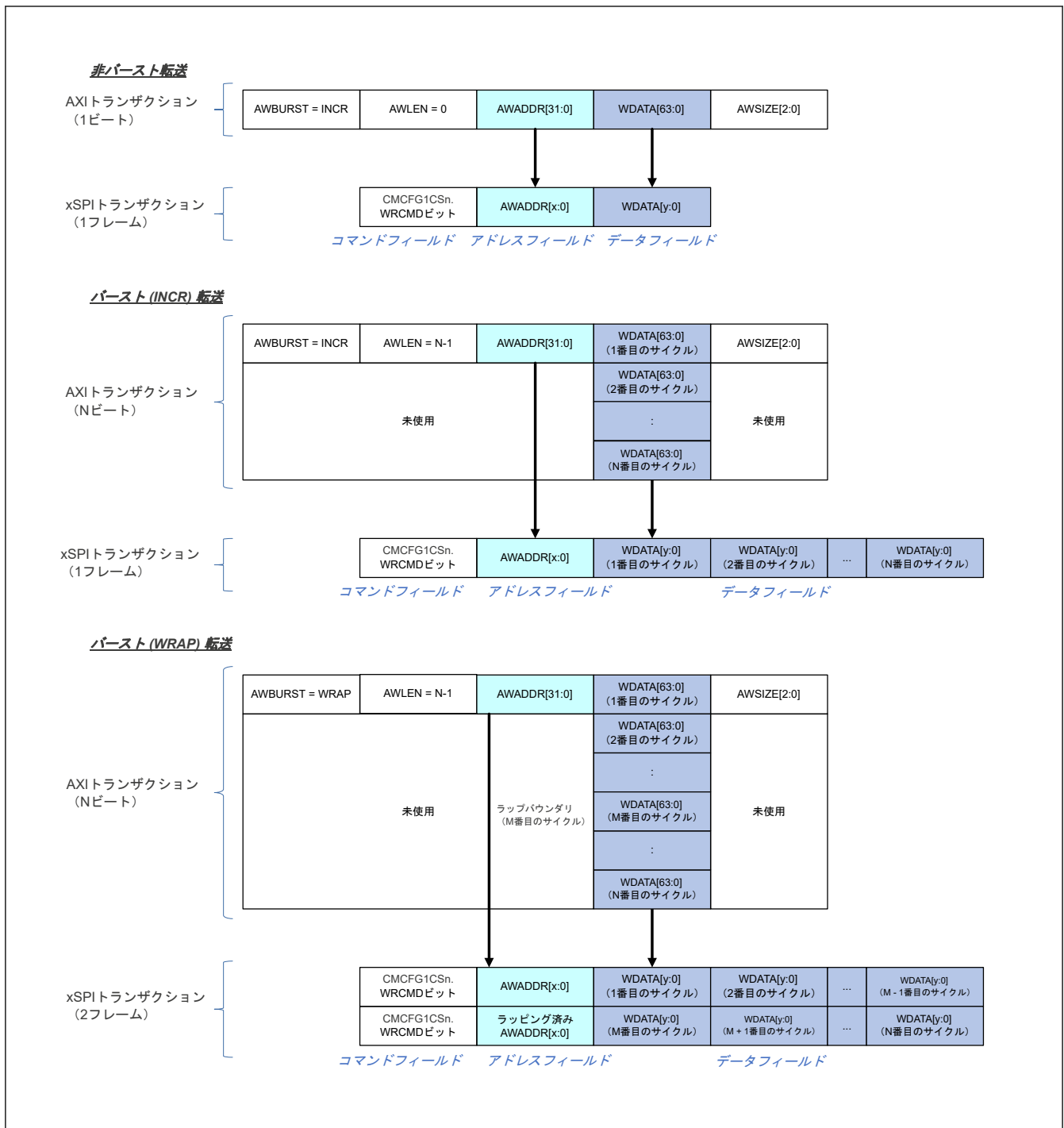
図 35.13 書き込みアクセス時の xSPI フレームのフォーマット (通常フォーマット)
