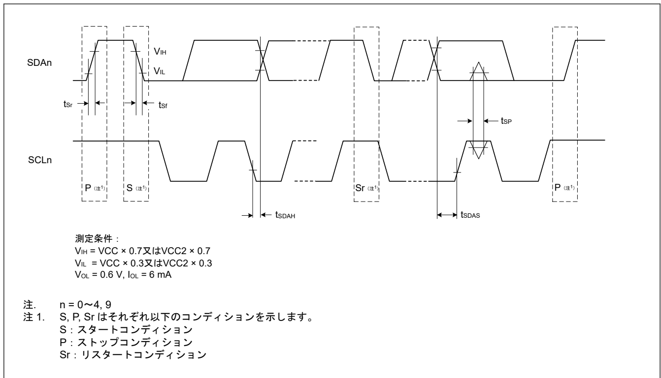
図 52.41 SCI 簡易 IIC モードタイミング
