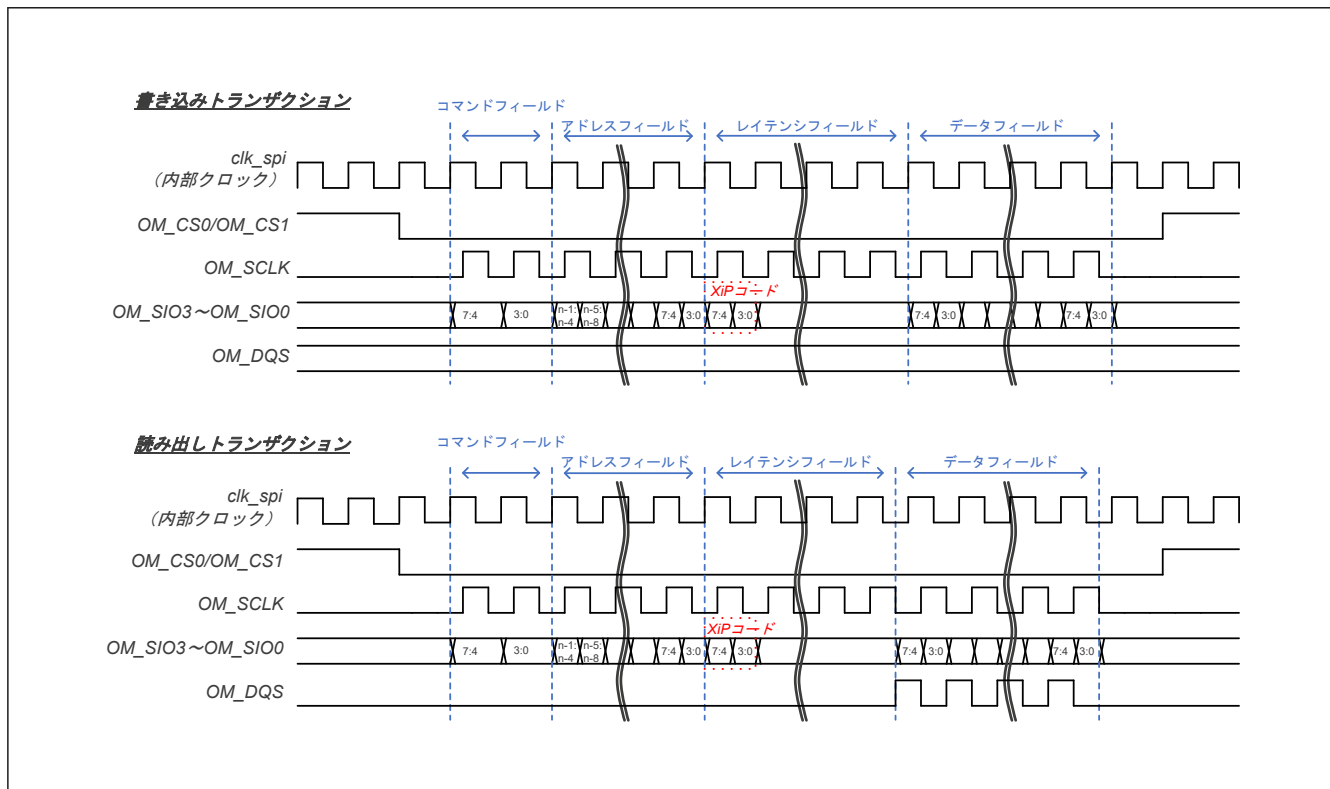
図 35.5 4S-4D-4D のタイミングチャート
