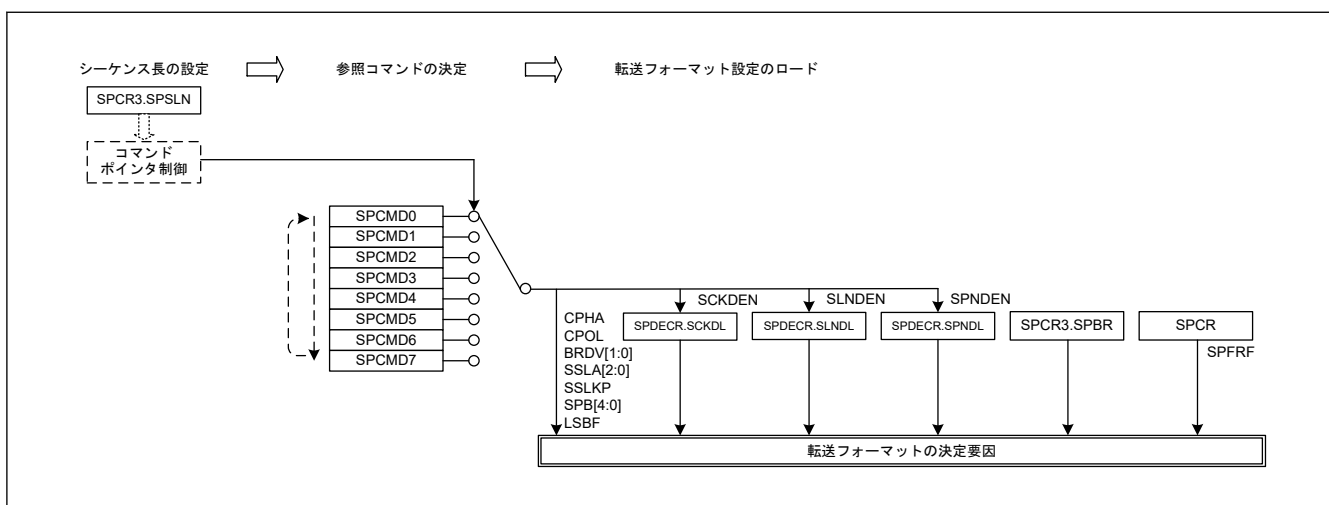
図 34.54 マスタモードでのシリアル転送方式の決定方法
