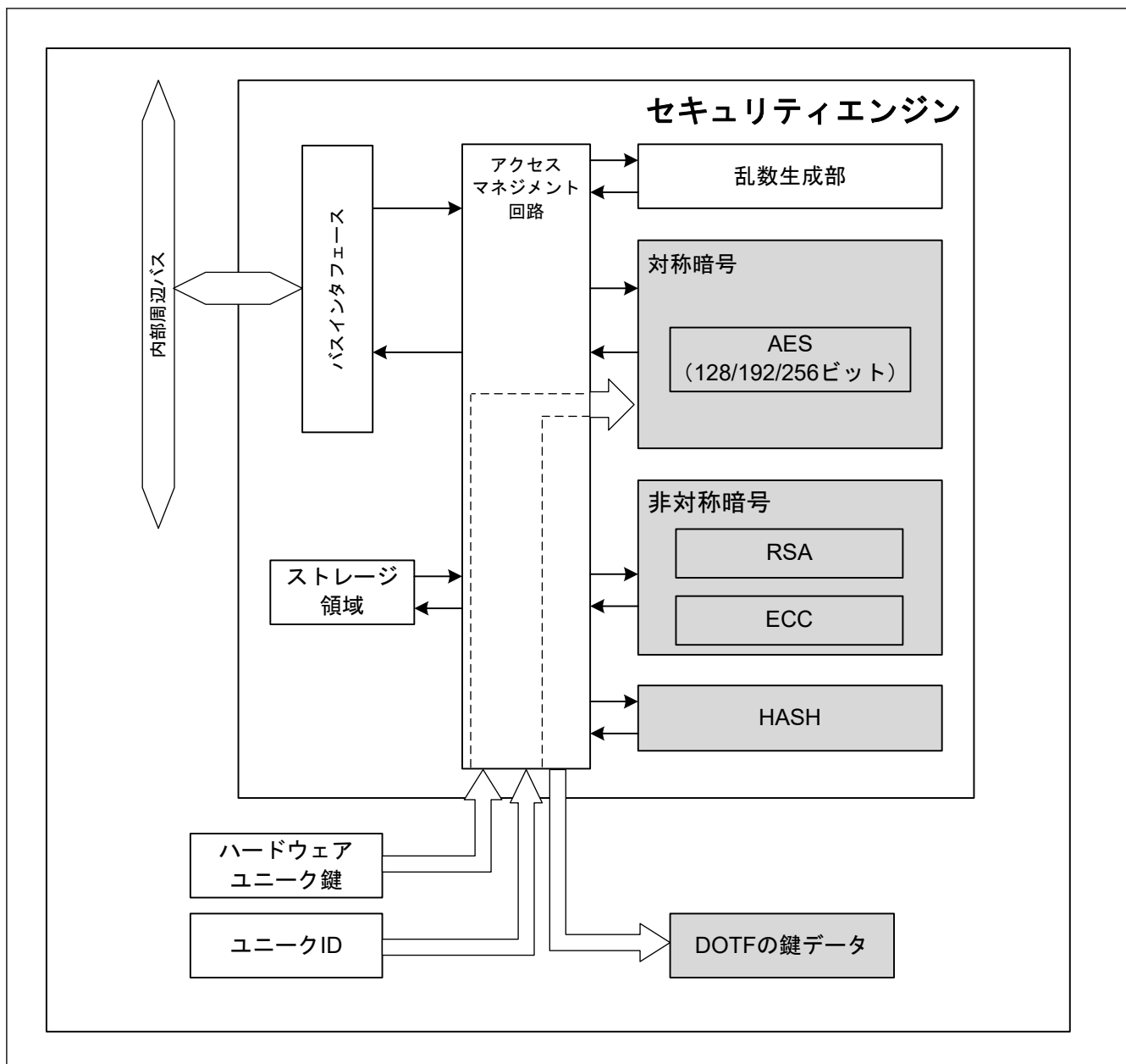
図 41.1 セキュリティエンジンのブロック図
