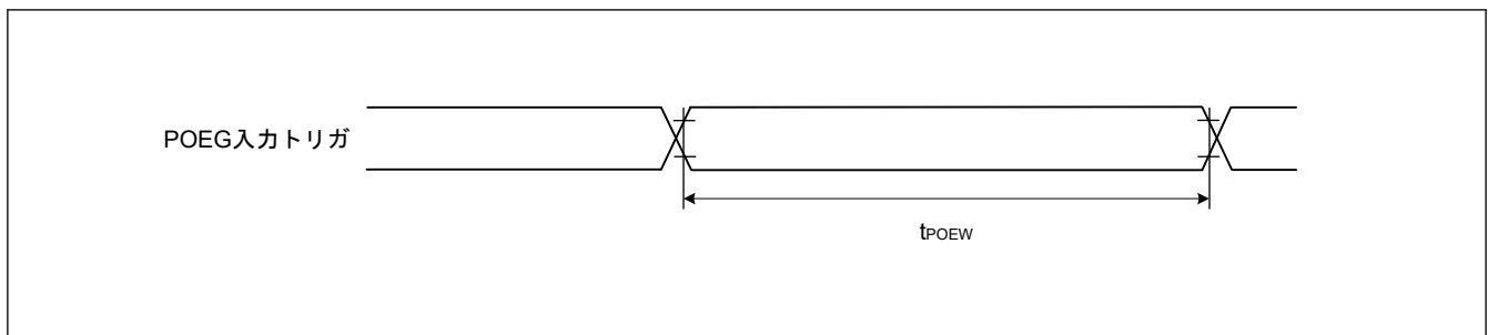
図 52.29 POEG 入力トリガタイミング
