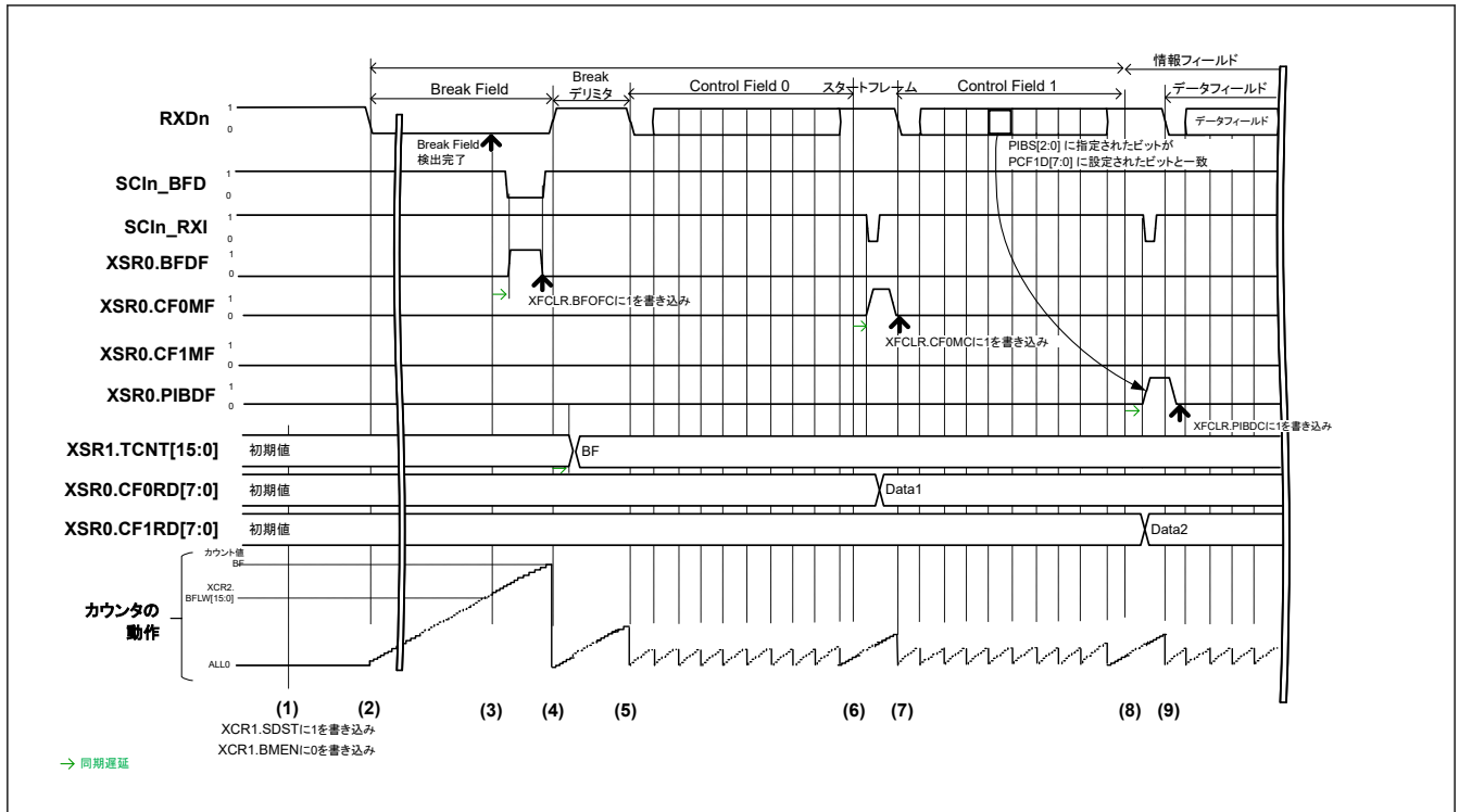
図 30.109 スタートフレーム受信例（優先割り込みビットを使用）
