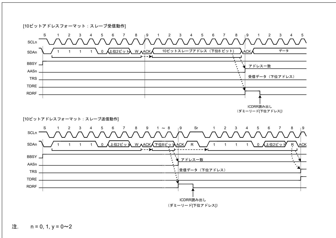
図 31.25 AASn フラグが1になるタイミング (10ビットアドレスフォーマット選択時)
