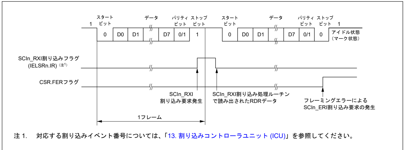
図 30.19 調歩同期式モードにおけるシリアル受信の動作例 (1) (RTS 機能を使用しない場合) (8 ビットデータ / パリティあり / 1 ストップビットの場合)
