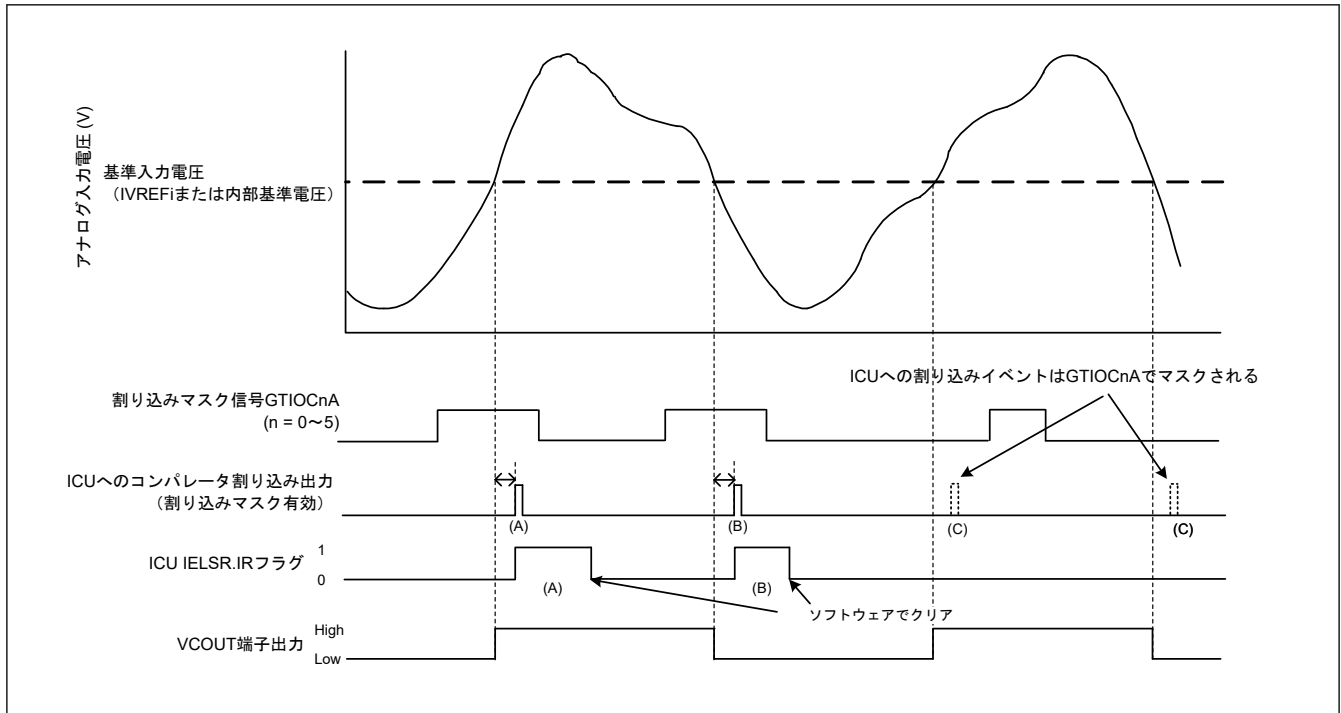
図 45.3 ACMPHS の動作例 (割り込みマスク機能有効)
