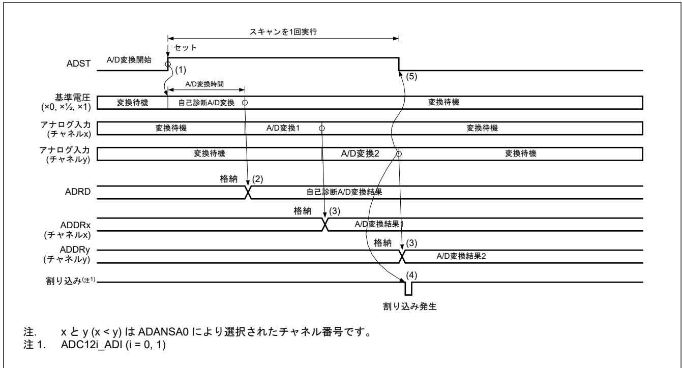
図 42.11 シングルスキャンモードの基本動作例（アナログ入力（チャンネル x、y）選択+自己診断）
