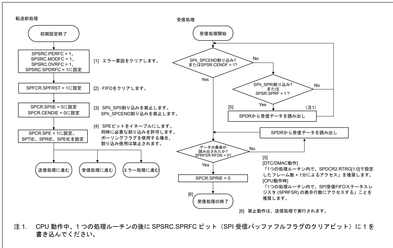
図 34.65 マスタモードでの受信手順
