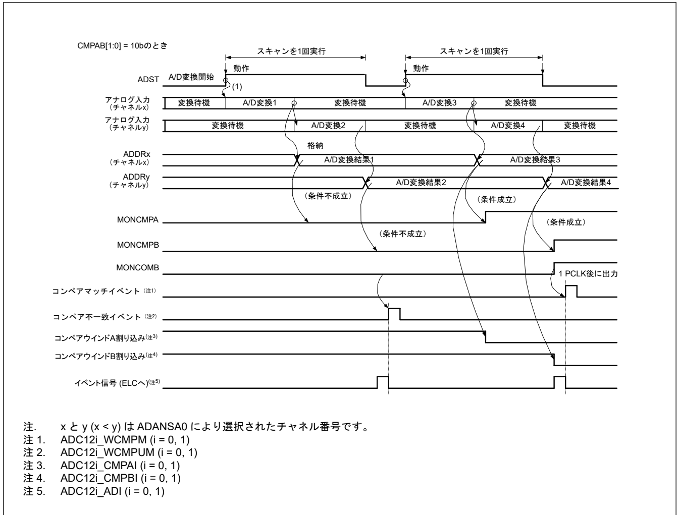
図 42.34 コンペア機能のイベント出力の動作例 (アナログ入力 (チャンネル x、y) を比較)
