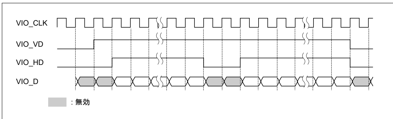
図 50.12 データイネーブ爾取り込みタイミング (VD が High の期間内に HD がアサート (High))
