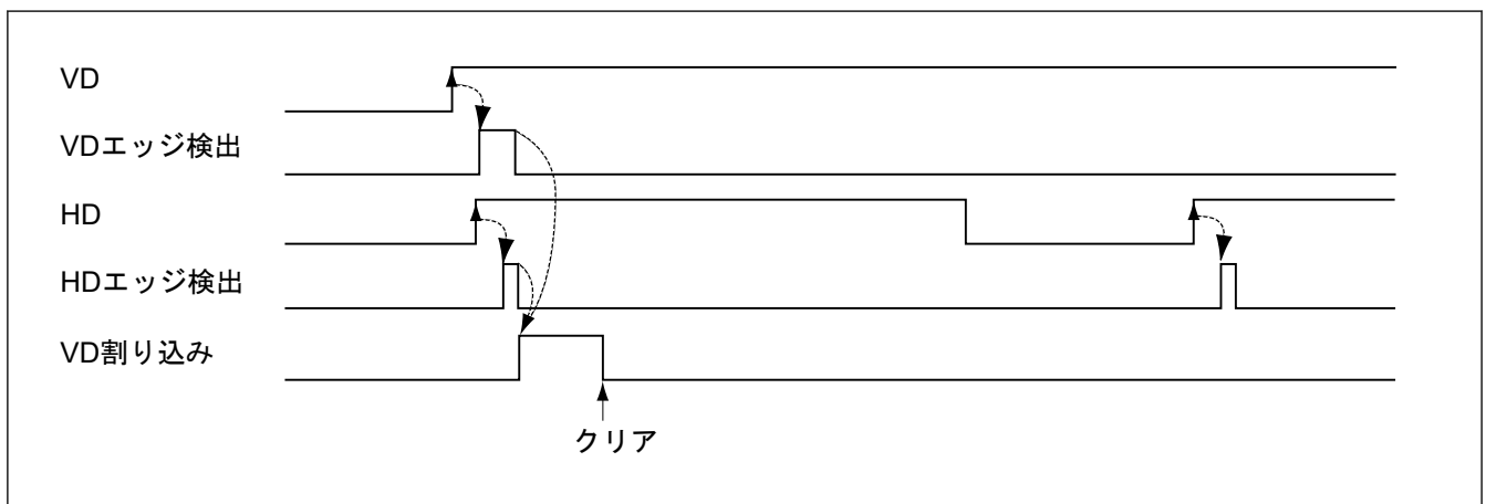
図 50.15 VD と HD が正極性の場合の VIO_VD および VIO_HD 信号と VD 割り込みの関係 (画像キャプチャモードおよびデータ同期取り込みモードの場合)
