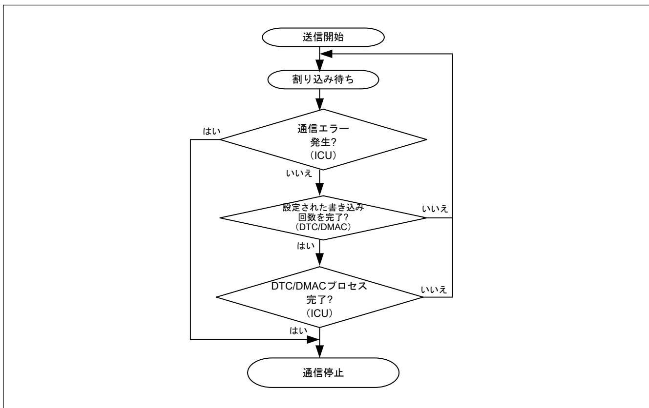
図 37.54 送信手順
