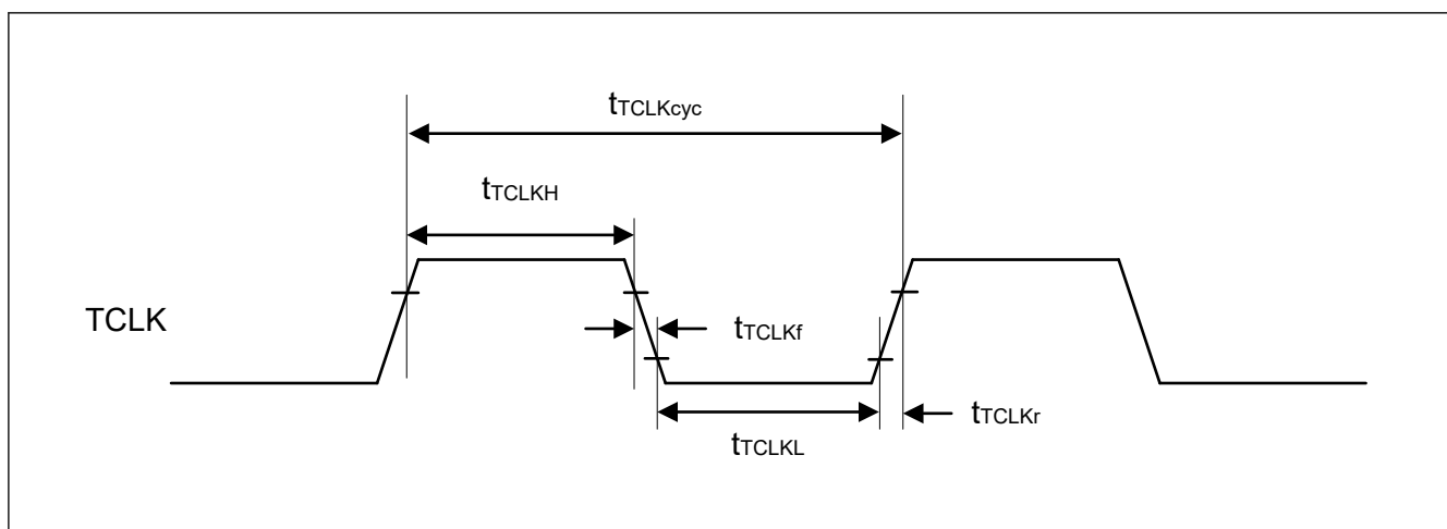
図 52.94 ETM TCLK タイミング
