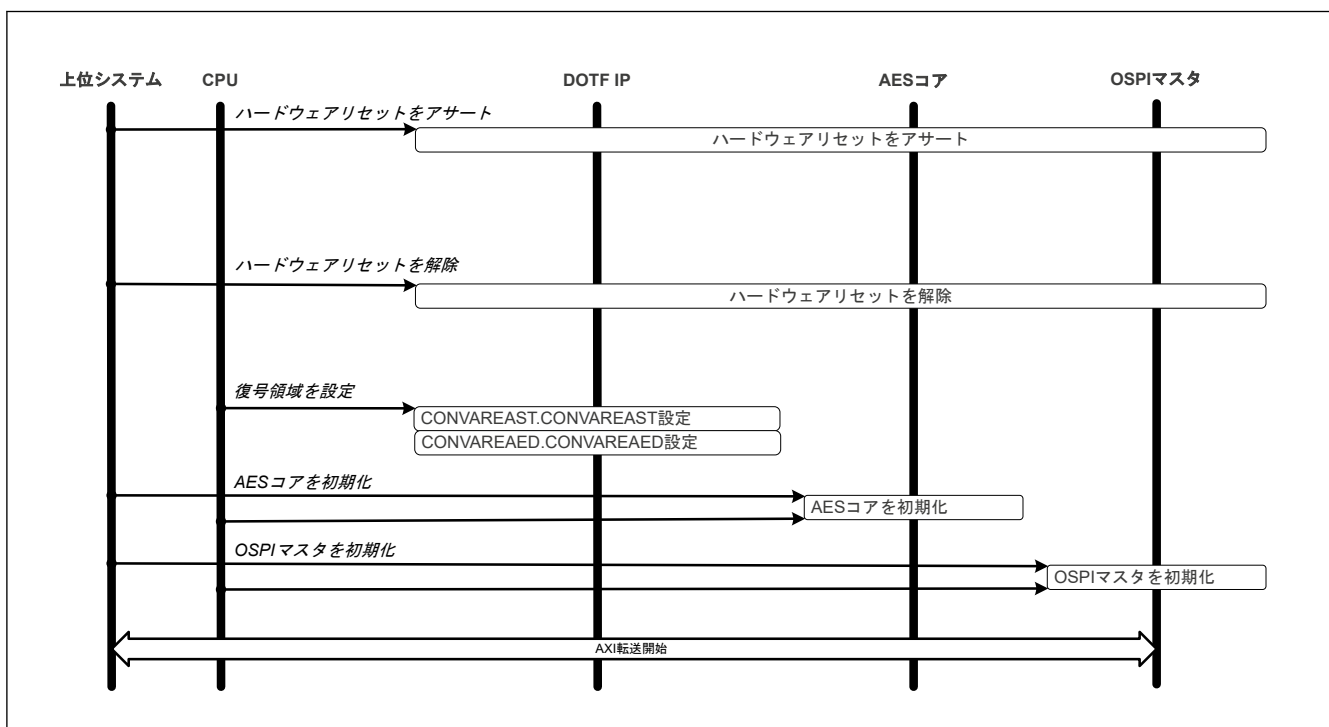
図 36.3 初期化フロー
