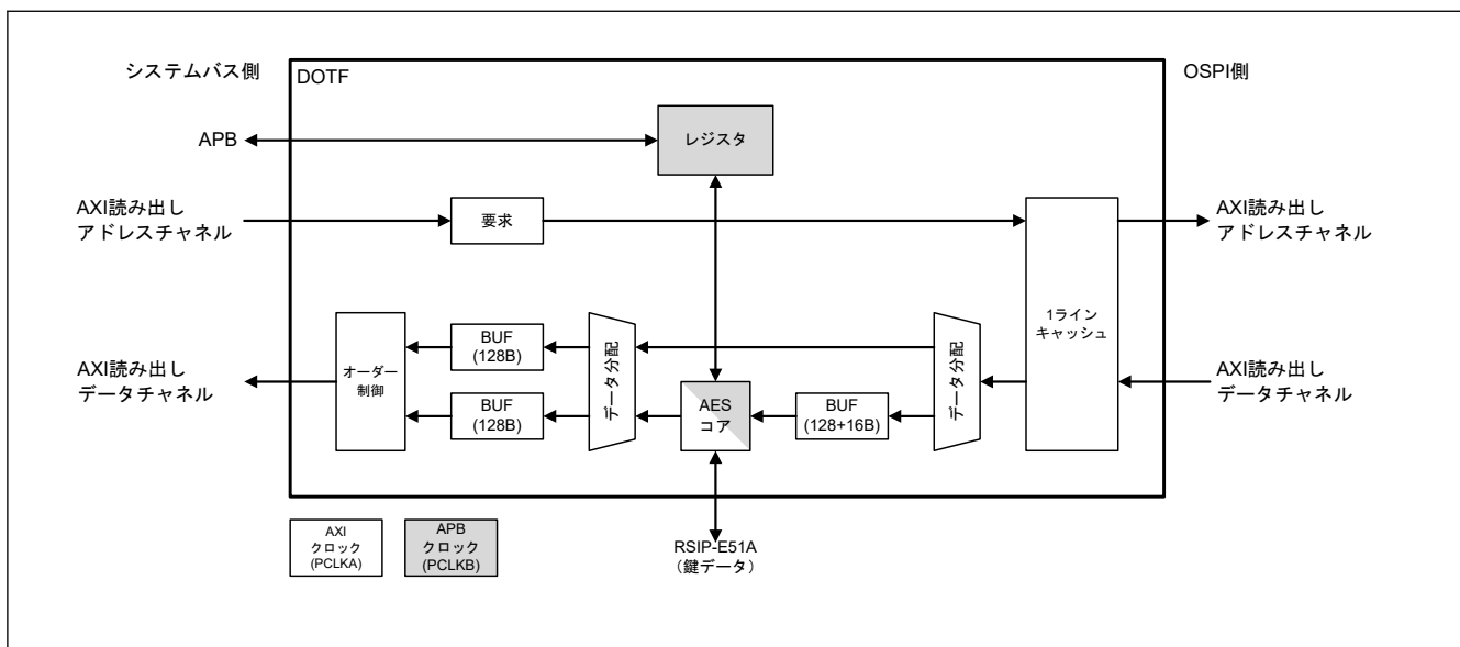
図 36.1 ブロック図
