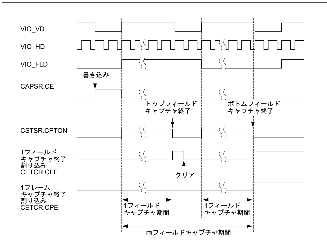
図 50.23 両フィールド画像キャプチャの1フレームキャプチャ終了割り込みおよび1フィールドキャプチャ終了割り込み
