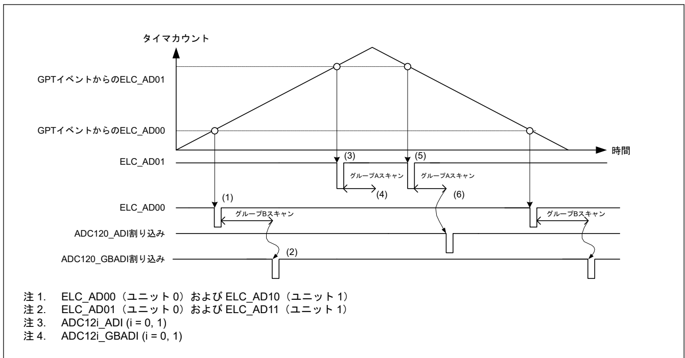
図 42.25 グループスキャンモードでダブルトリガモードを使用する場合の基本動作例 (ELC からの同期トリガ使用時)
