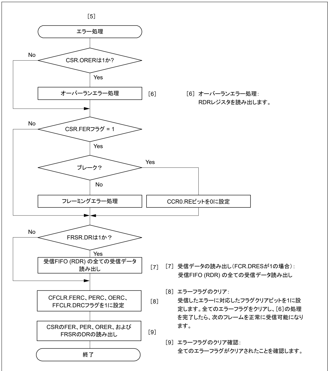
図 30.44 マルチプロセッサモードにおけるシリアル受信のフローチャート例 (2) (FIFO 選択時)
