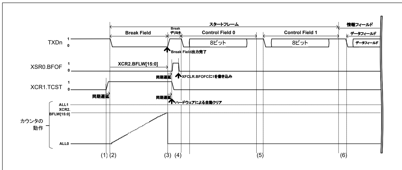
図 30.102 スタートフレーム送信例
