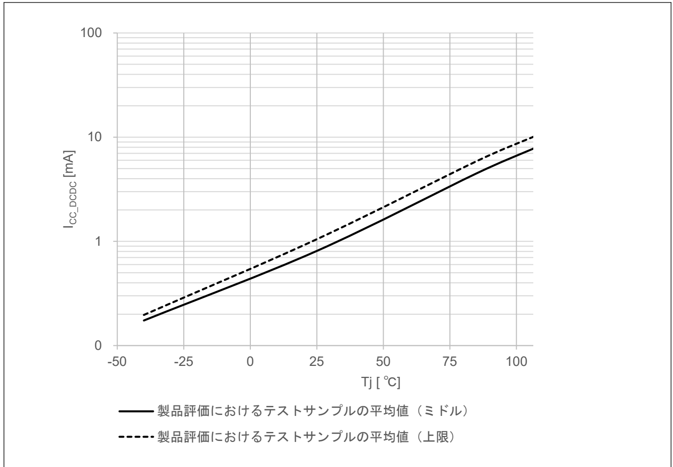
図 52.4 ソフトウェアスタンバイモードにおける温度依存性 ( I_{cc\_DcDc} ) (参考データ)
