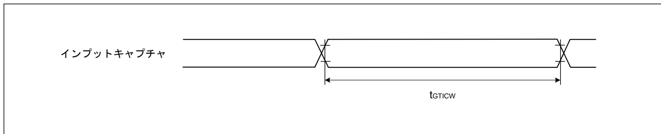
図 52.30 GPT インプットキャプチャタイミング
