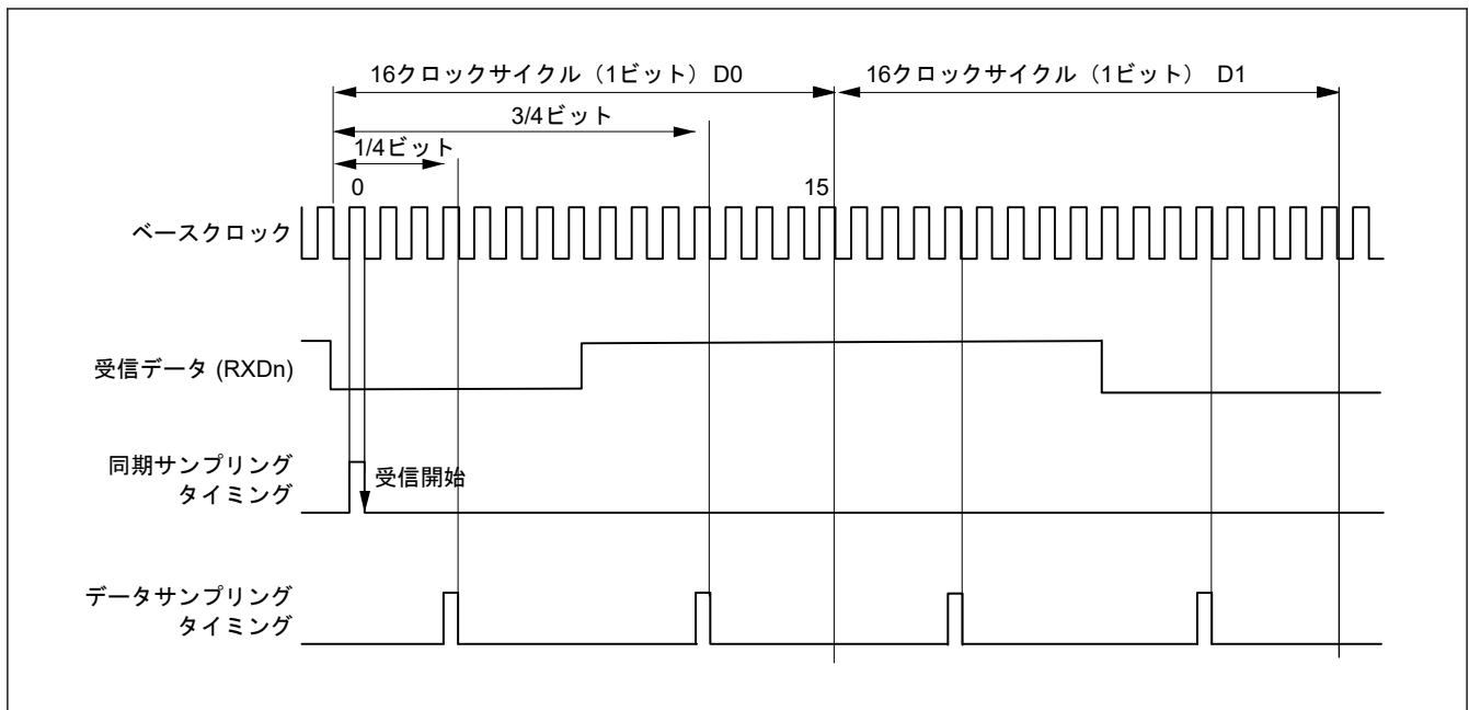
図 30.55 マンチェスタモードでのデータ受信サンプリングタイミング
