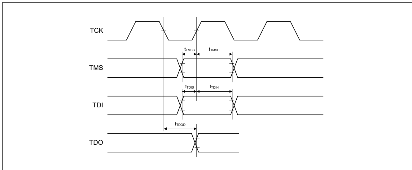
図 52.87 バウンダリスキャン入出力タイミング (1)
