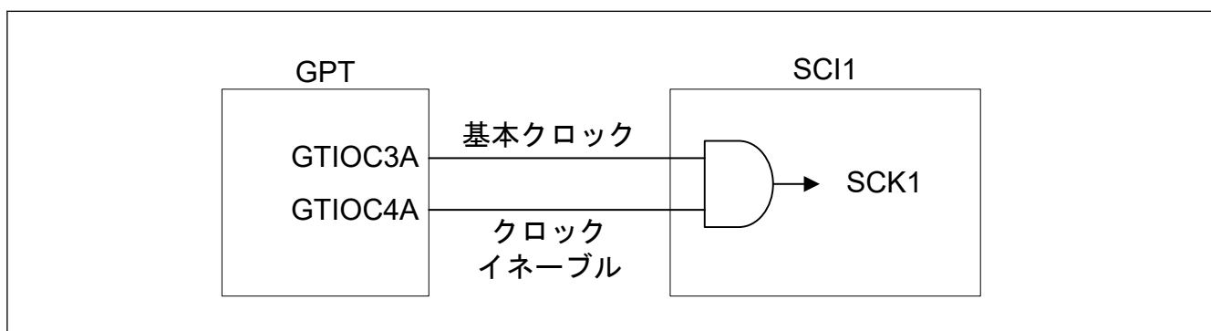
図 30.4 GPT と SCI の接続例
