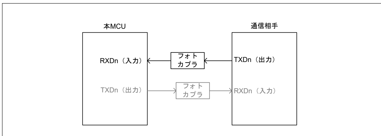
図 30.26 フォトカプラを通過する受信のブロック図イメージ
