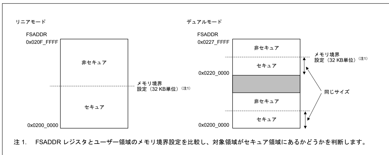
図 49.39 ユーザー領域内のセキュア領域と非セキュア領域 (セキュアエイリアスの場合)
