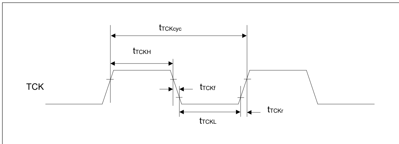
図 52.90 JTAG TCK タイミング
