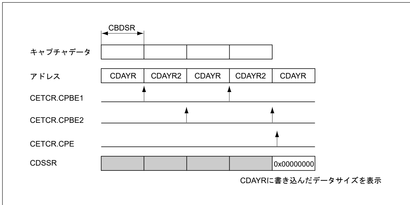
図 50.48 バンドル書き込み時の CDSSR 動作タイミングイメージ図 (バンドル書き込み終了とキャプチャ終了が同時の場合)
