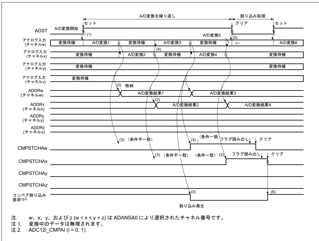
図 42.32 コンペア機能の動作例 (アナログ入力 (チャンネル w~z) を比較)
