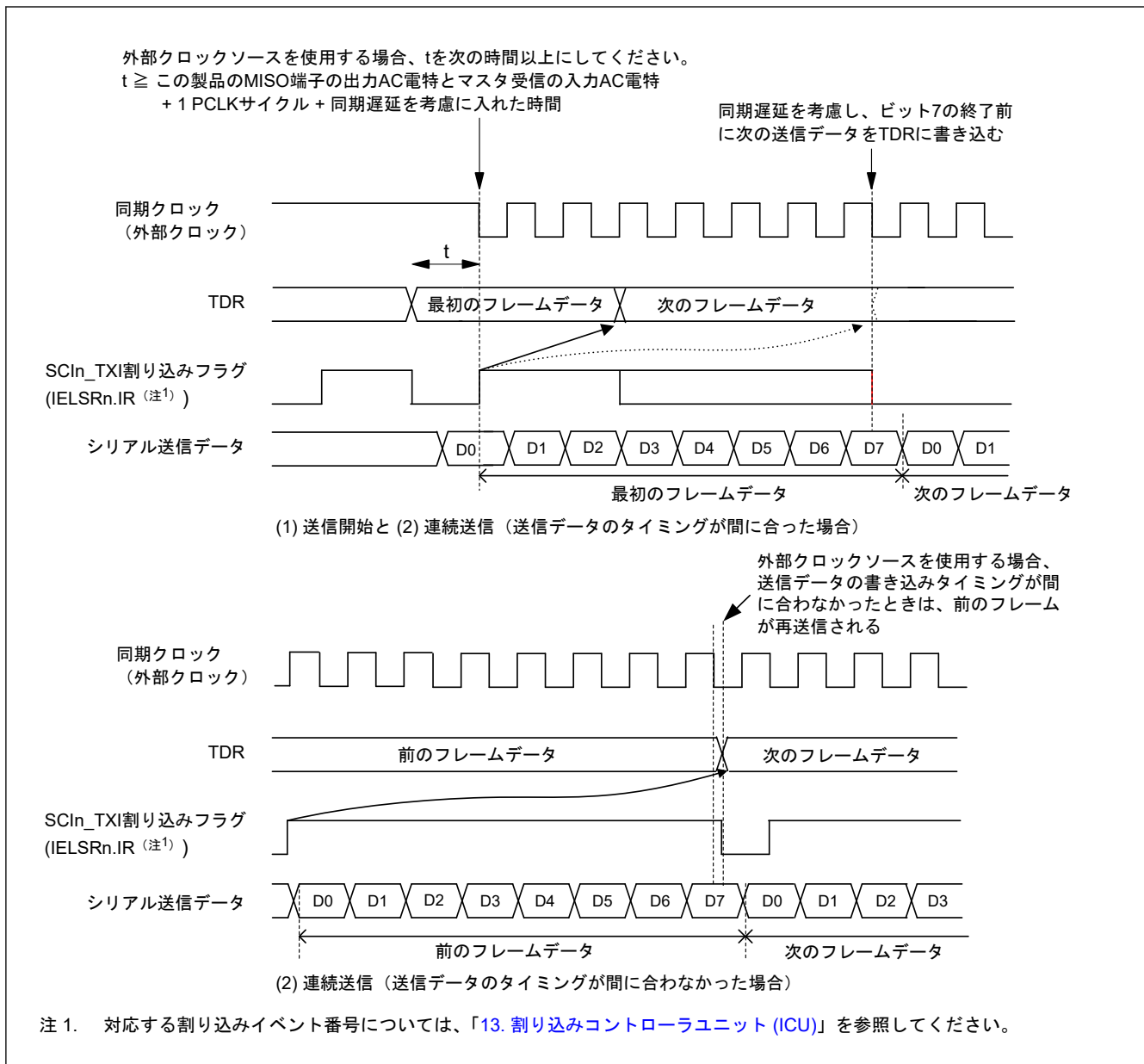
図 30.121 クロック同期式送信時の外部クロック使用に関する制約事項
