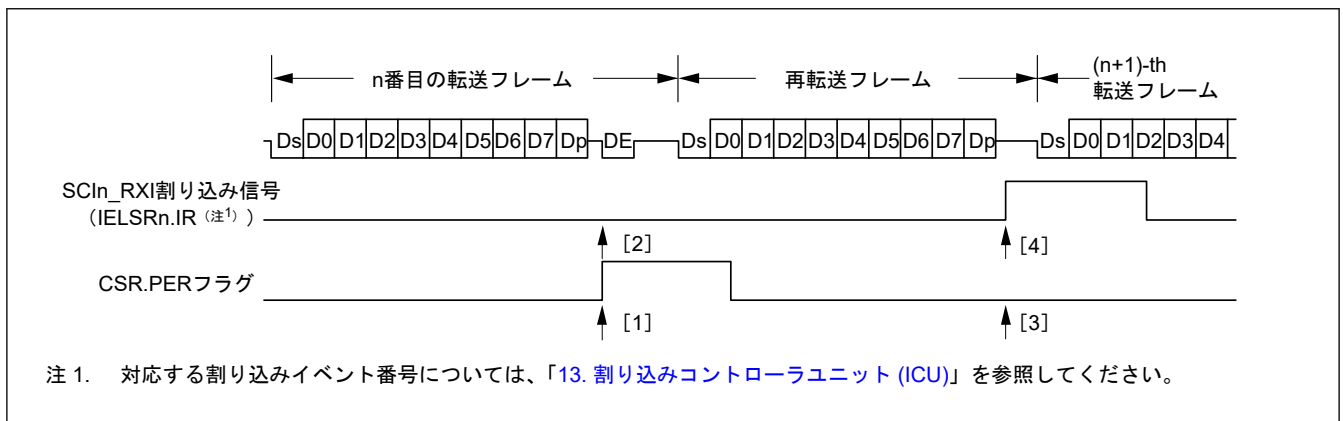
図 30.83 スマートカードインタフェース受信モードでの再転送動作
