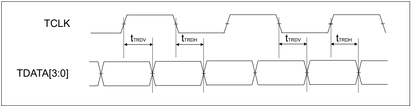
図 52.95 ETM 出力タイミング
