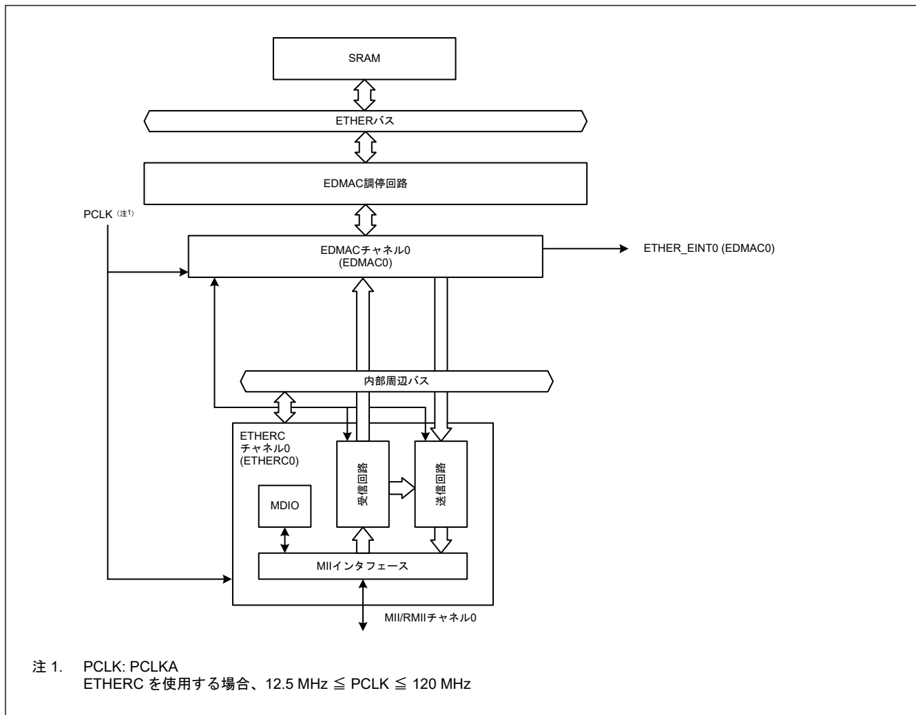
図 27.1 ETHERC 構成
