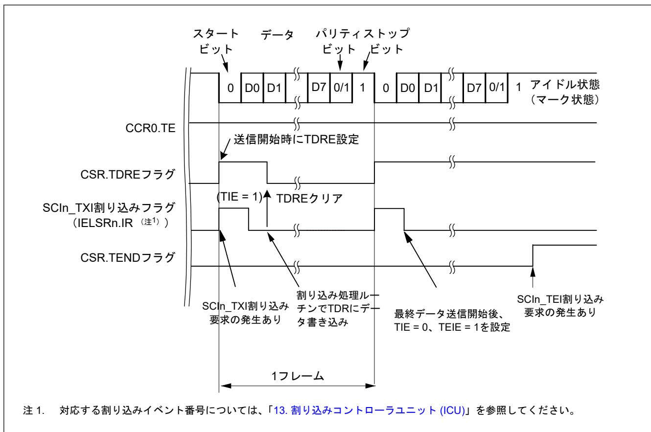
図 30.14 調歩同期式モードにおけるシリアル送信の動作例 (3) (8 ビットデータ/パリティあり/1ストップビット/CTS 機能不使用/送信途中~送信完了時)
