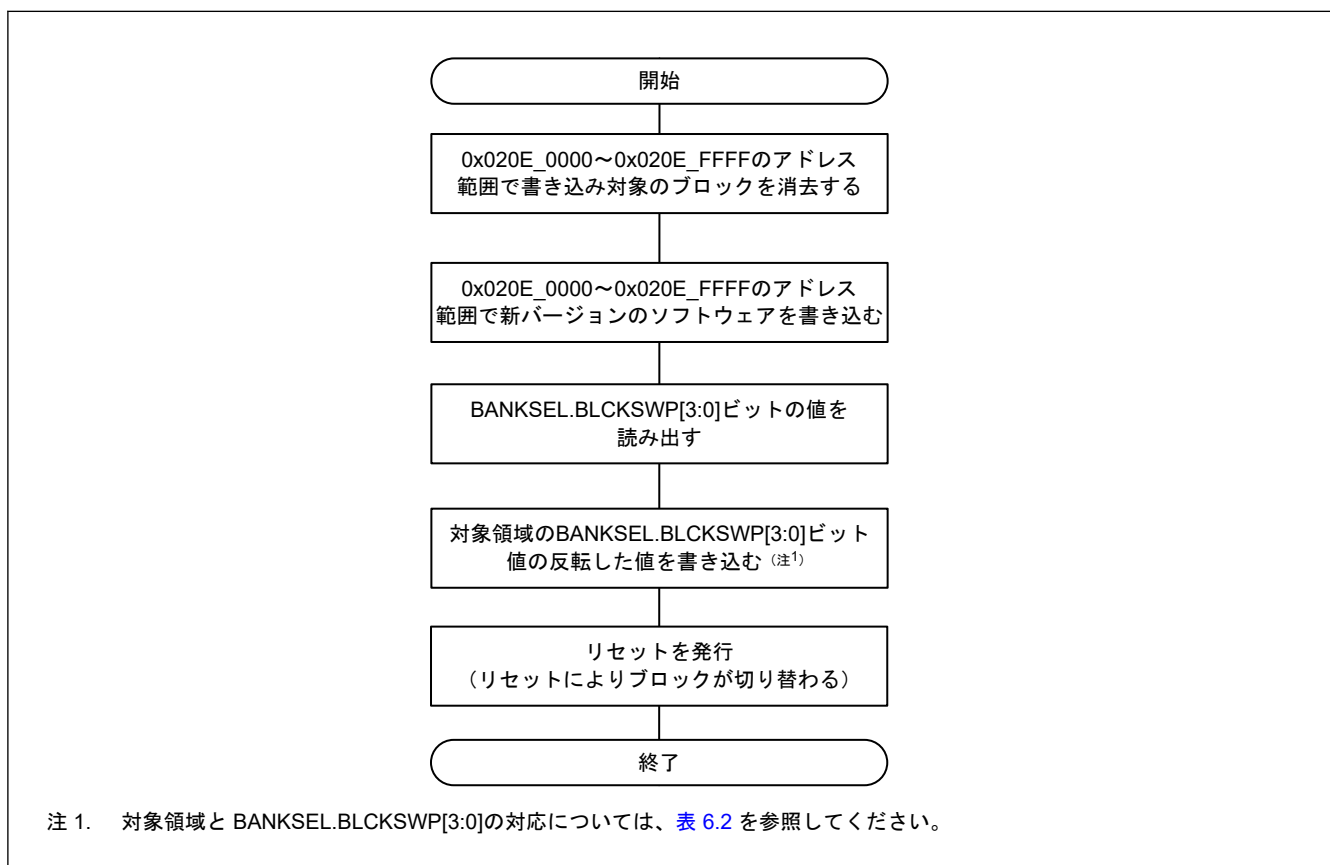
図 49.36 ブロックスワップ選択フロー例 (セキュアエリアの場合)
