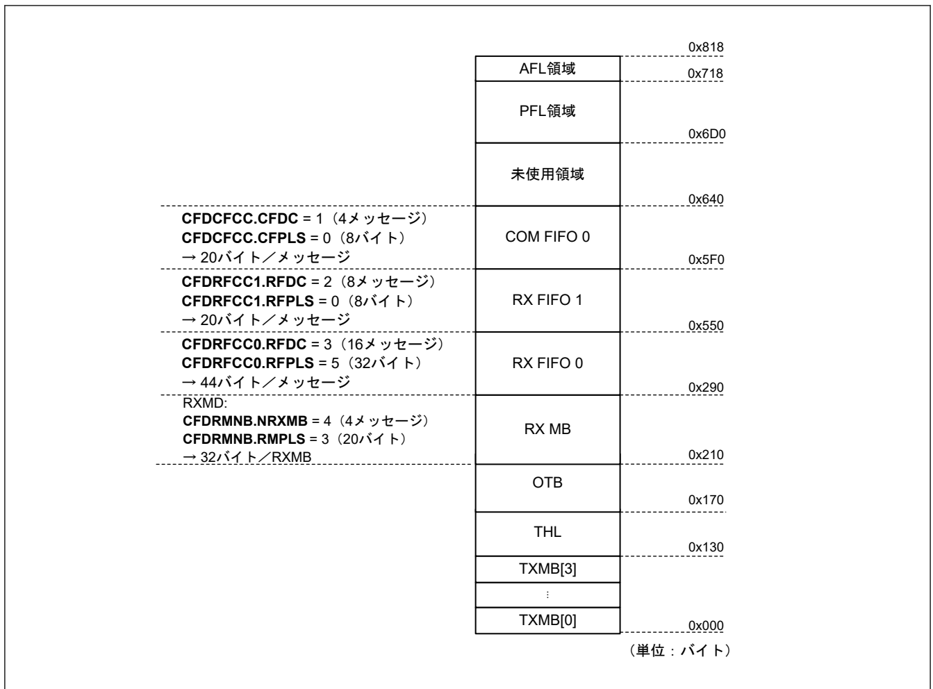
図 32.55 RX MB + FIFO バッファの RAM 領域の構成例
