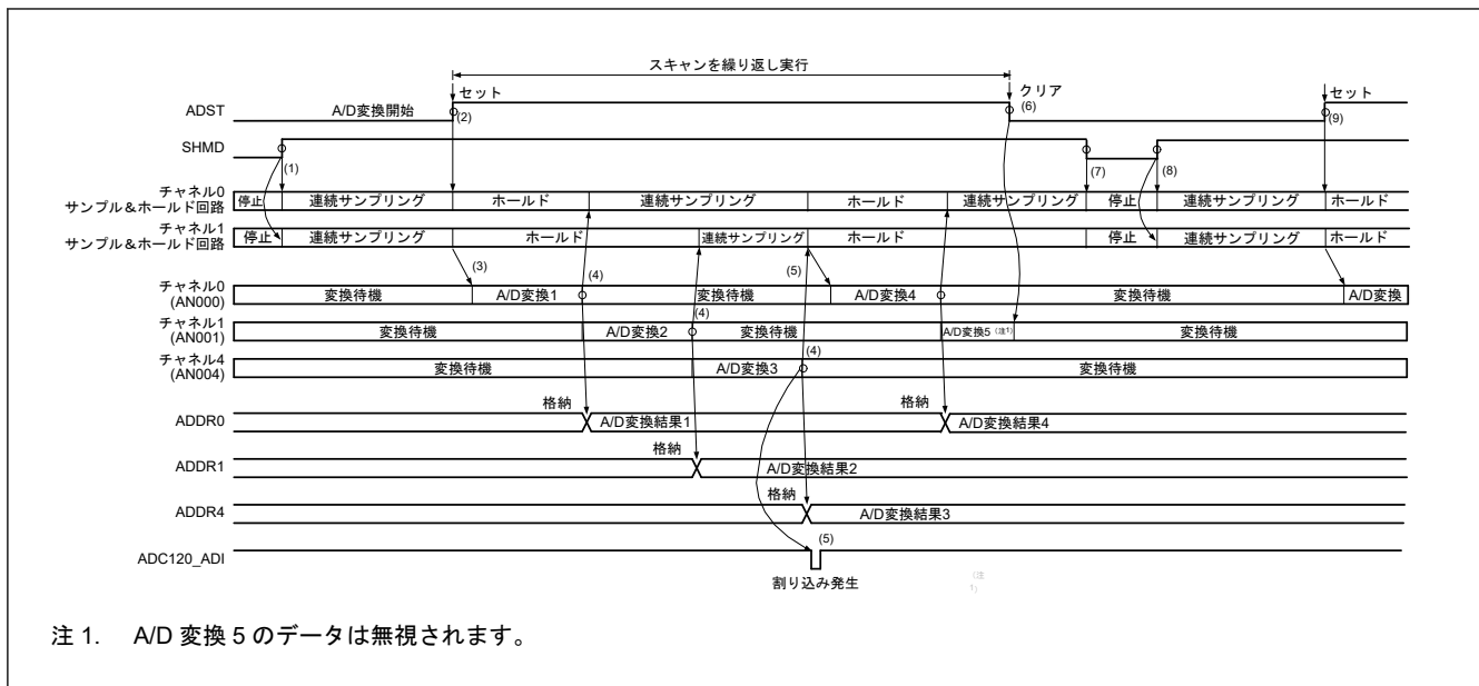
図 42.19 連続スキャンモードの動作例 (チャンネル専用サンプル&ホールド回路使用、AN000、AN001、および AN004 選択、連続サンプリング有効)
