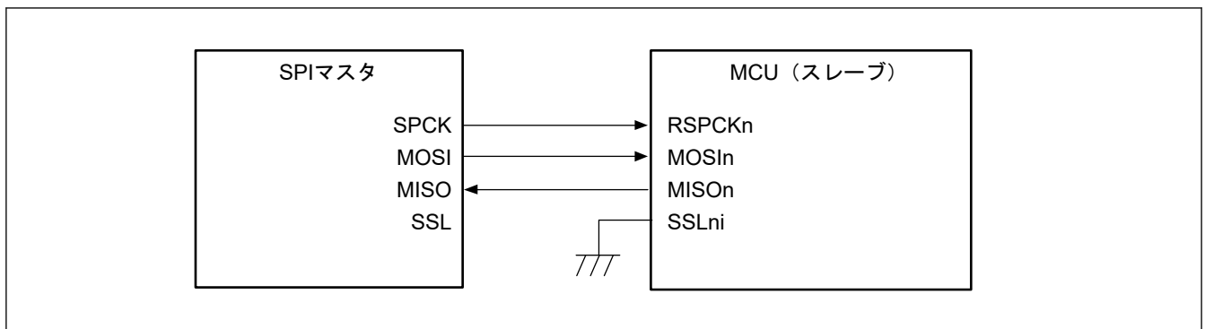
図 34.8 シングルマスタとシングルスレーブの構成例 (MCU はスレーブ、SPCMDm.CPHA = 1)
