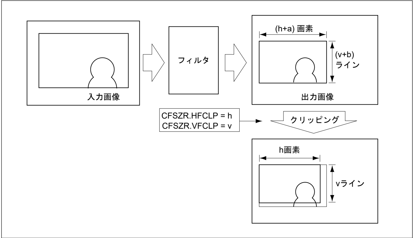
図 50.33 フィルタ出力画像のクリッピング
