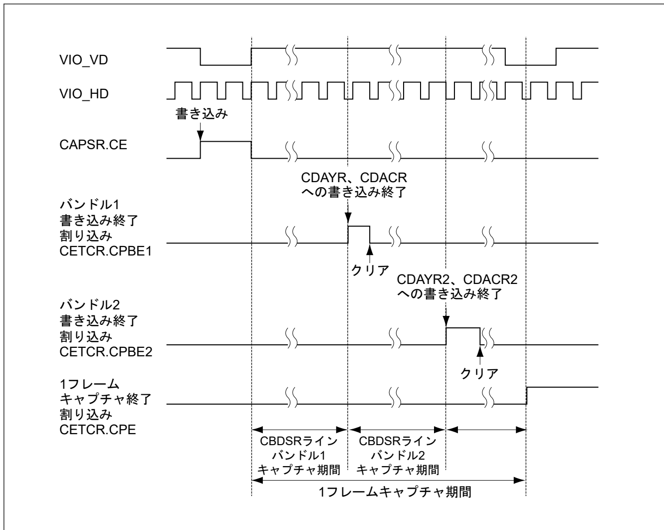
図 50.42 書き込み終了割り込みのタイミング (画像キャプチャ時、データ同期取り込み時)
