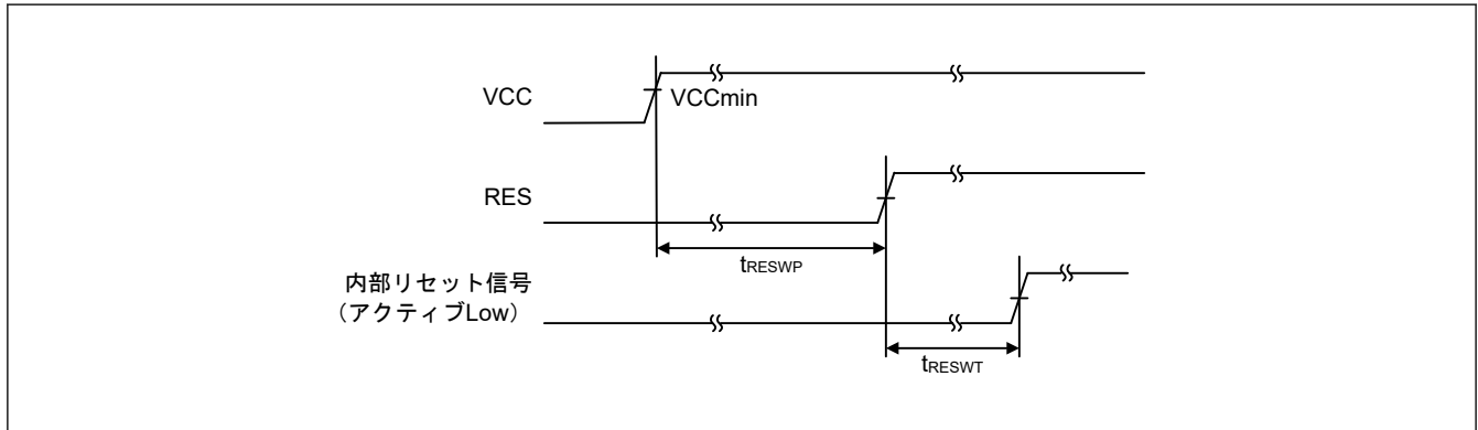
図 52.21 VCC が V POR 電圧しきい値を超える条件下での RES 端子入力タイミング
