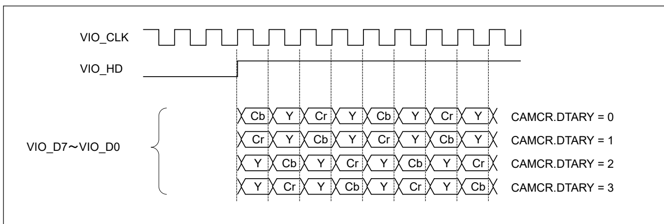
図 50.11 画像データの入力順序
