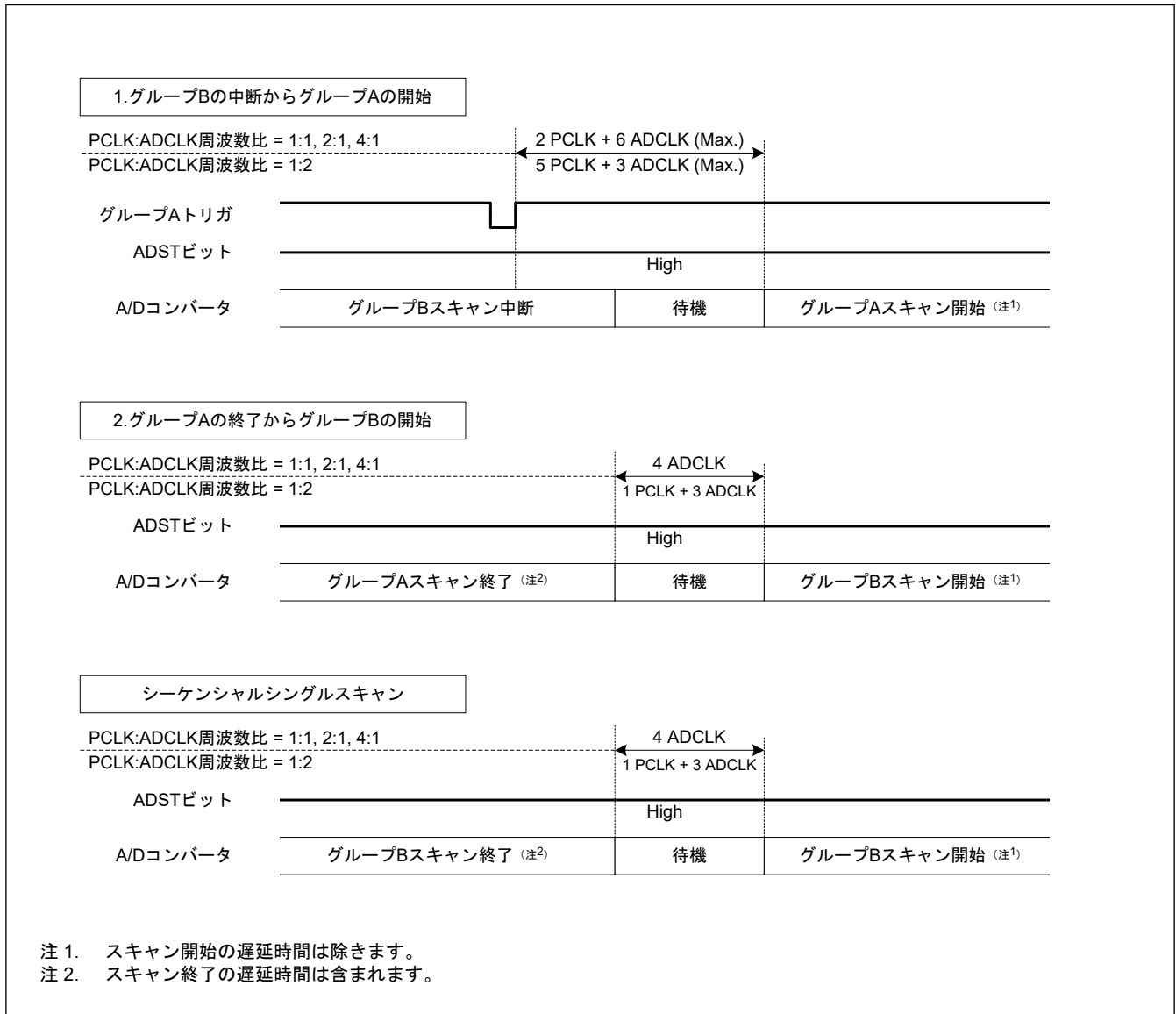
図 42.37 グループ優先制御における動作でのスキャンの中断/開始タイミング図
