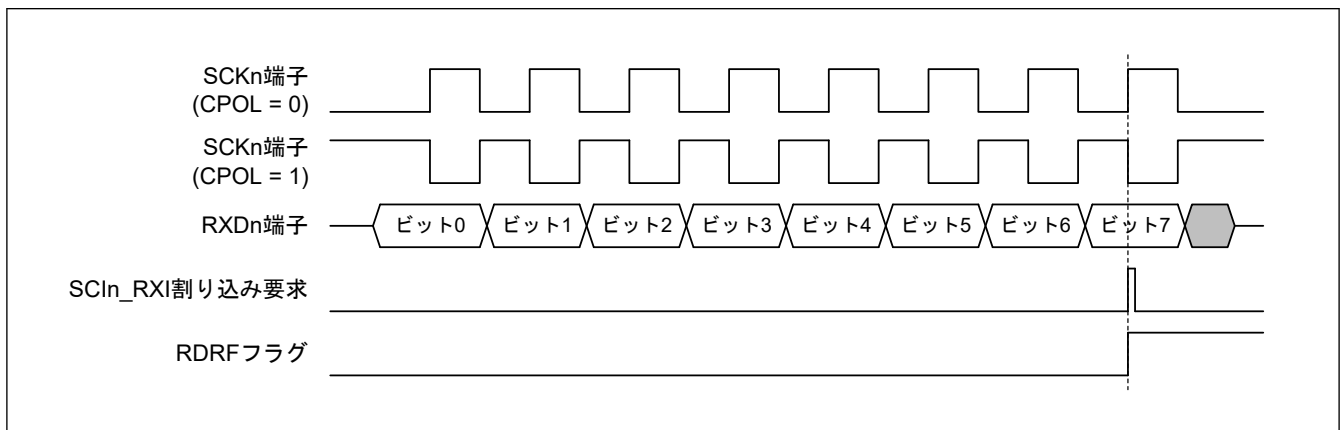
図 30.122 簡易 SPI モードにおける SCI n _RXI 割り込みの発生タイミング (クロック遅れあり)
