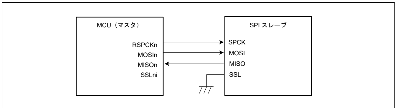
図 34.6 シングルマスタとシングルスレーブの構成例 (MCU はマスタ)
