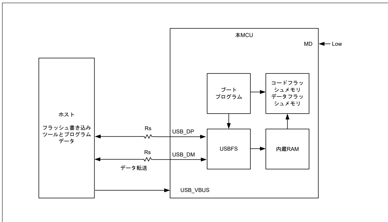
図 49.48 ブートモード (USB インタフェース) のシステム構成図
