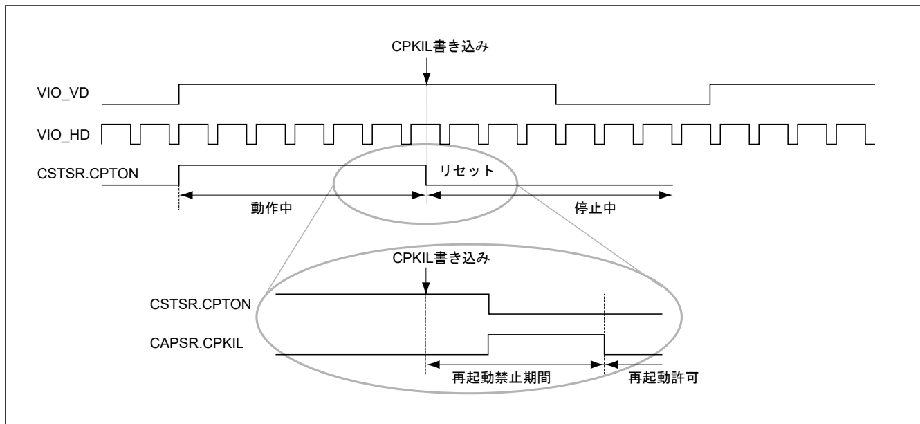
図 50.6 キャプチャのソフトウェアリセットおよび再起動のタイミング
