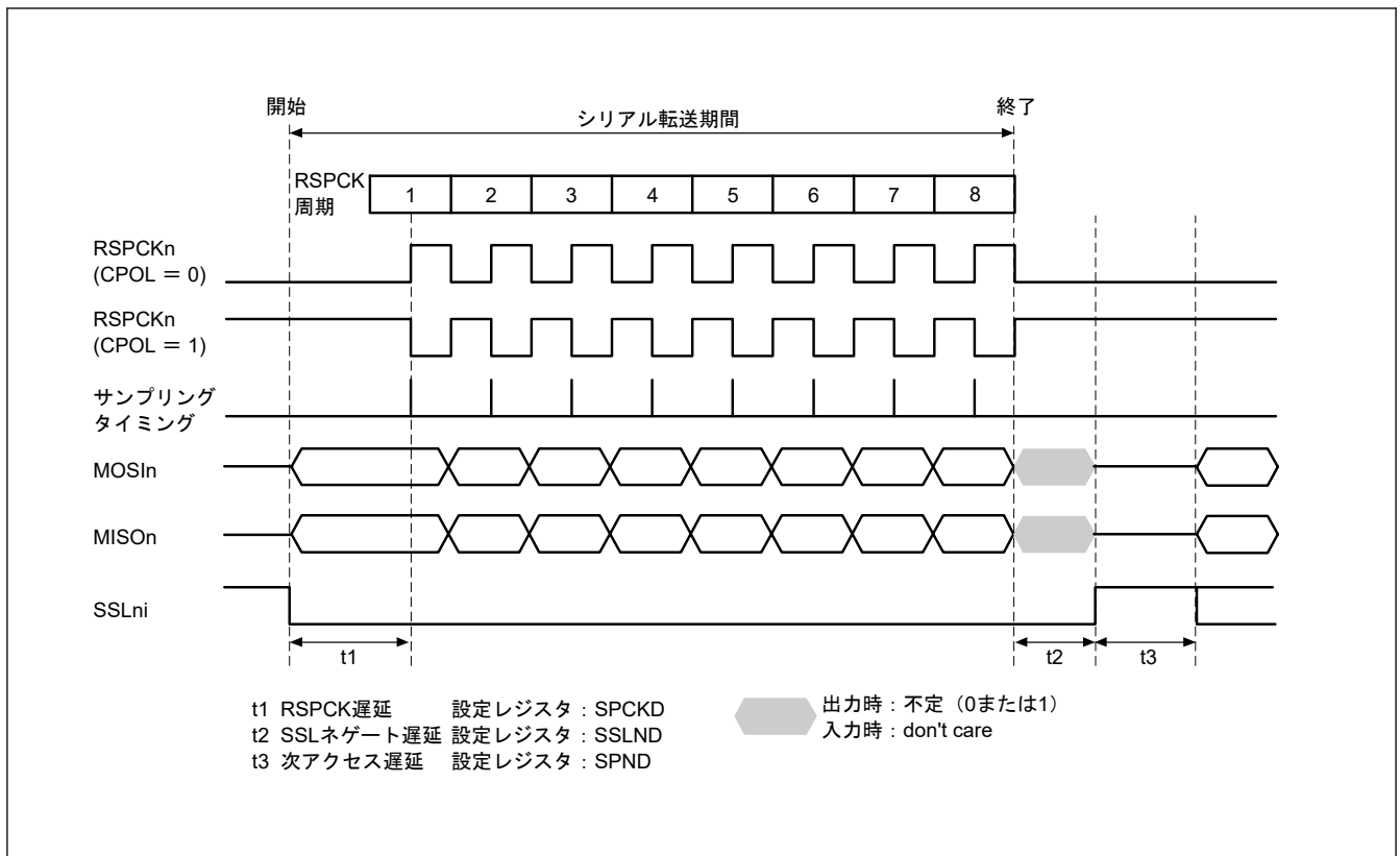
図 34.27 CPHA = 0、SPFRF = 0 の場合の SPI 転送フォーマット
