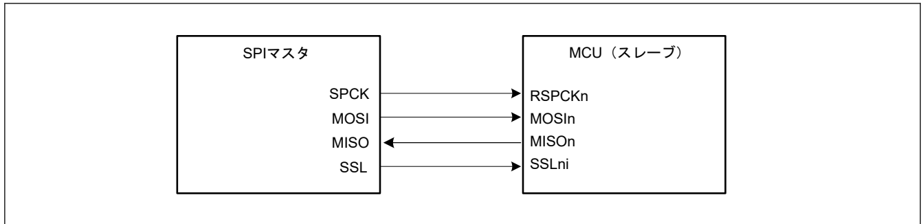
図 34.7 シングルマスタとシングルスレーブの構成例 (MCU はスレーブ、SPCMDm.CPHA = 0)
