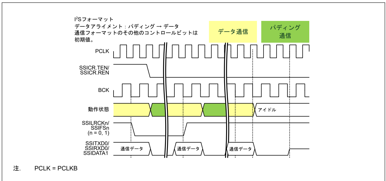
図 37.50 データ通信からの停止（パディングビットあり）
