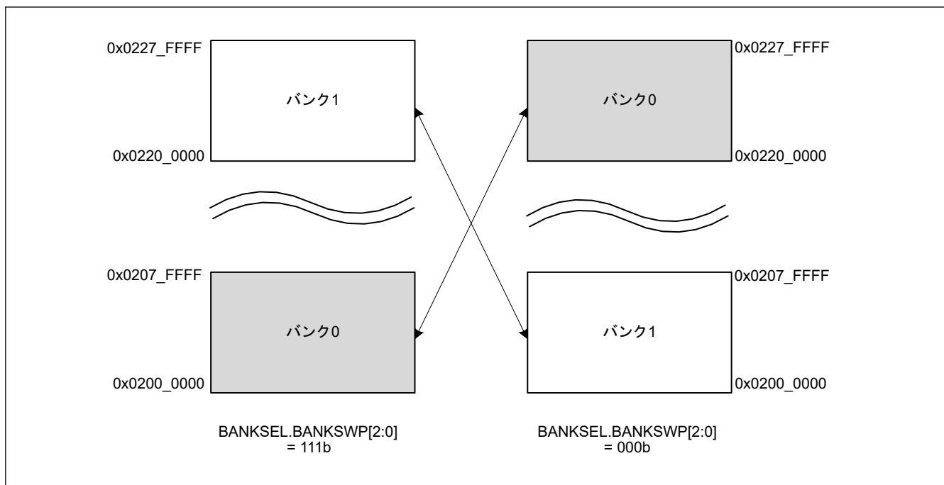
図 49.34 スタートアップバンク選択例（セキュアエリアの場合）
