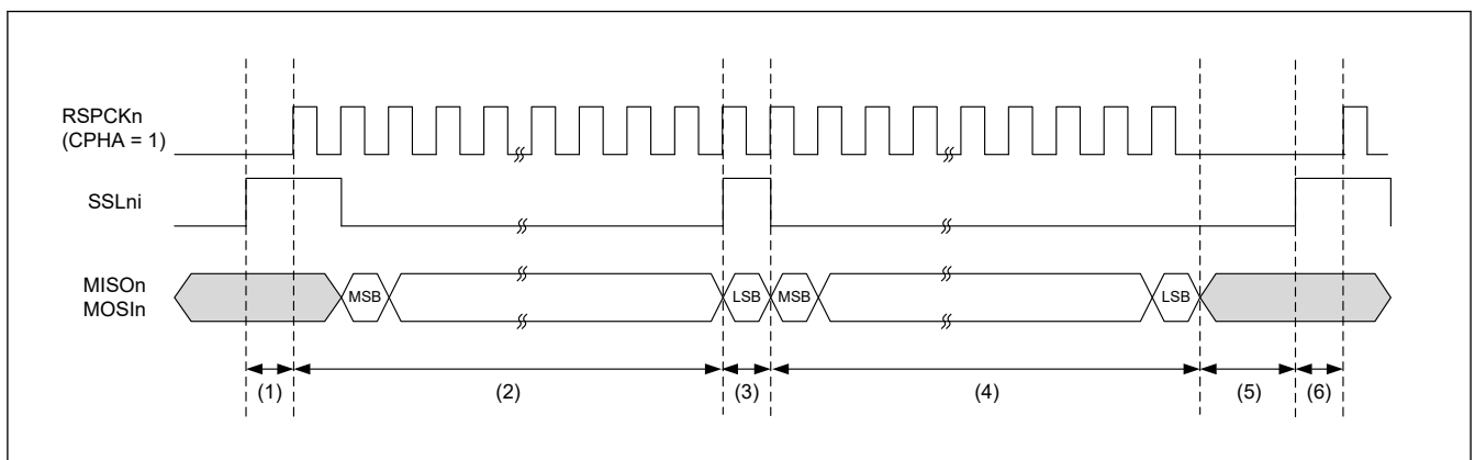
図 34.59 バースト転送の動作例 (SPFRF = 1)
