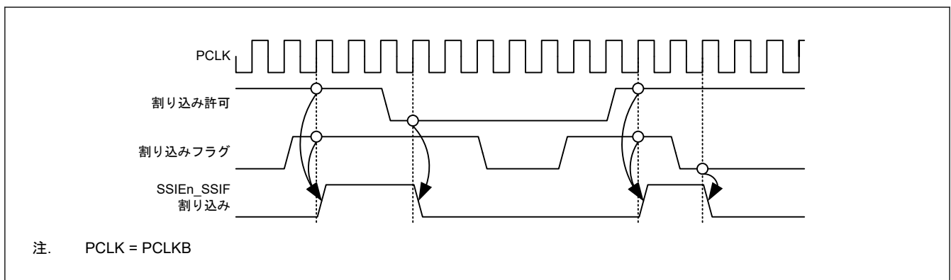
図 37.59 共通割り込み要因のタイミング図 (SSIEn_SSIF)
