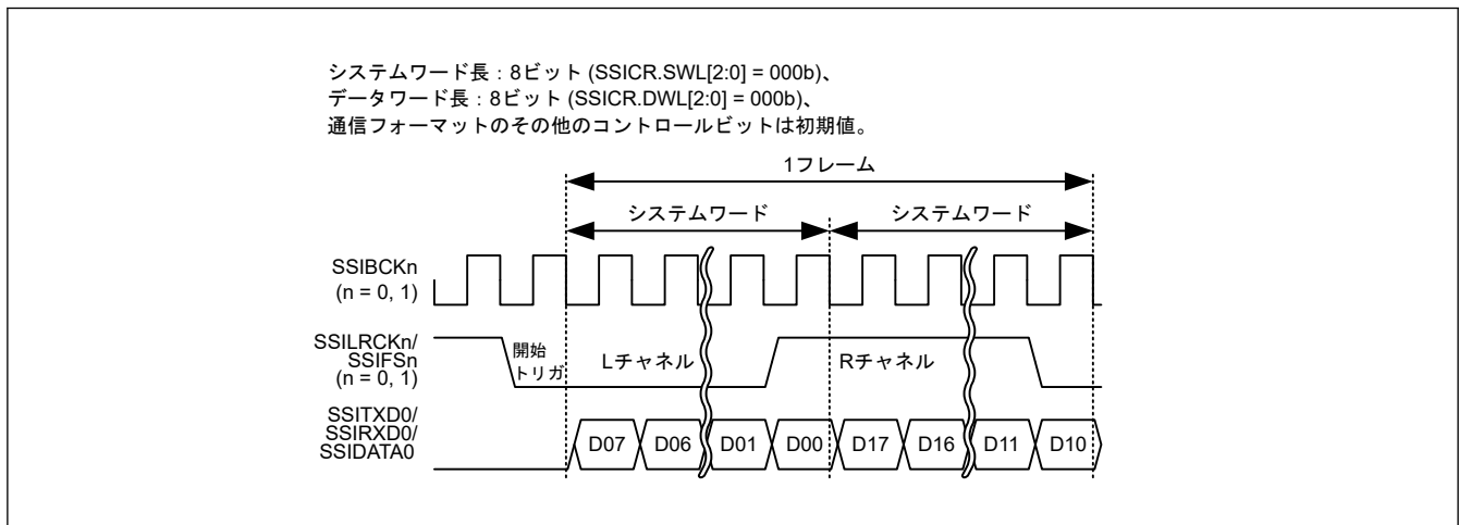
図 37.37 I 2 S フォーマット (パディングなし、システムワード長 = データワード長)
