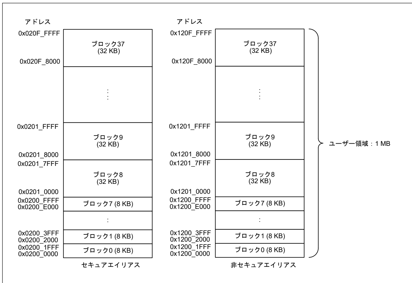
図 49.2 リニアモードでのコードフラッシュメモリのマップ
