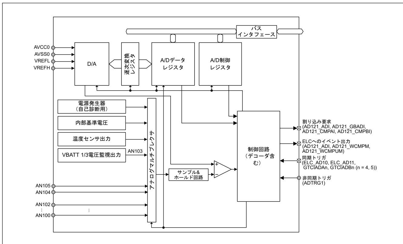
図 42.2 ADC12 のブロック図 (ユニット 1)
