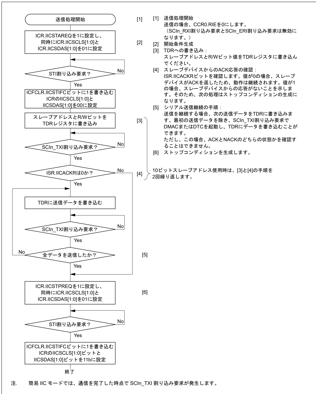
図 30.93 簡易 IIC モードにおけるマスタ送信のフローチャート例 (送信割り込み、受信割り込み使用時)
