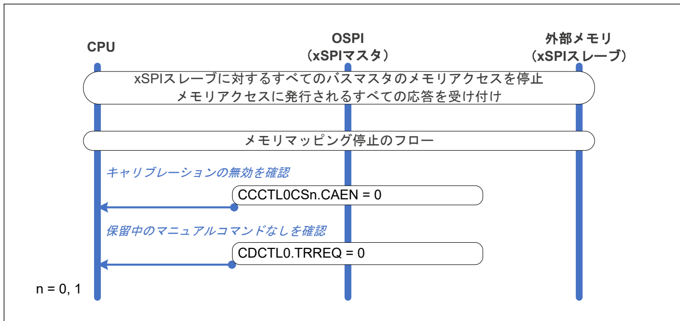
図 35.23 通信停止のフロー
