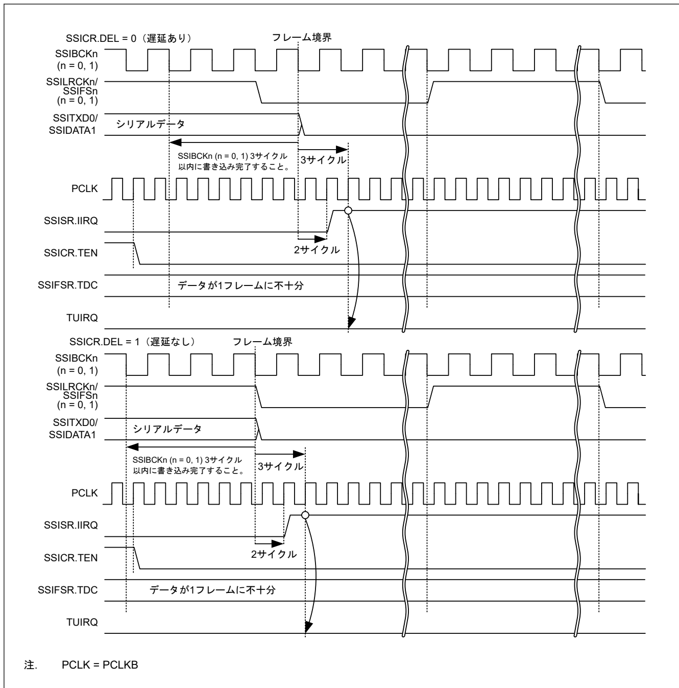
図 37.21 TUIRQ 設定タイミング (通信中断時)
