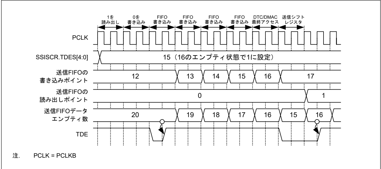
図 37.29 TDE の設定およびクリアに関するタイミング図
