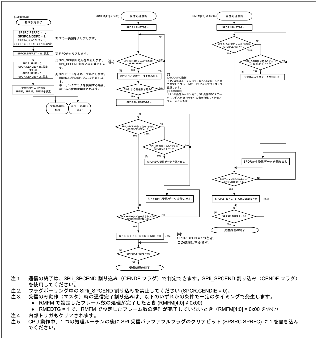
図 34.66 マスタモード時のソフトウェア処理フローチャート (受信のみ)
