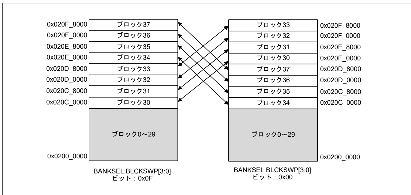
図 49.35 ブロックスワップ選択例 (セキュアエリアの場合)
