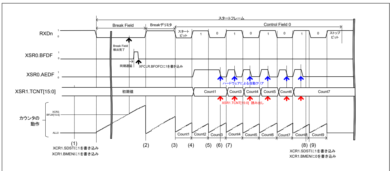
図 30.112 ビットレート測定機能の動作例
