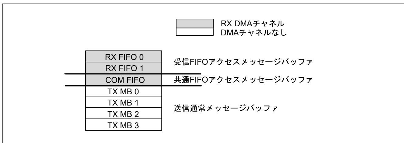
図 32.32 DMA チャンネルに接続可能なメッセージバッファ
