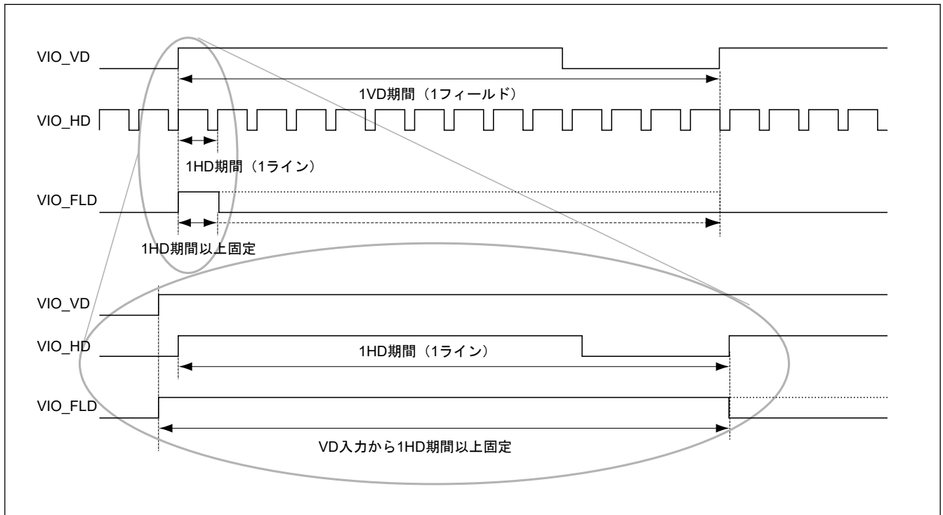
図 50.4 1 フィールドのタイミング
