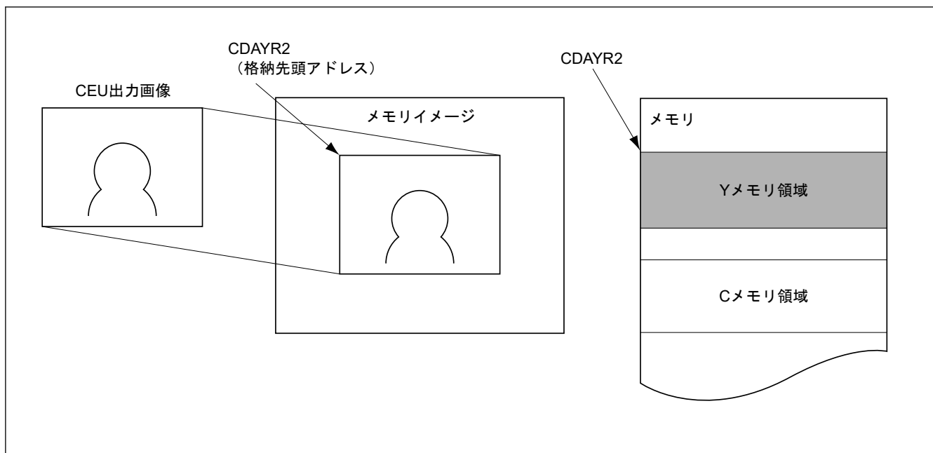
図 50.50 キャプチャ画像と輝度成分メモリ領域の関係
