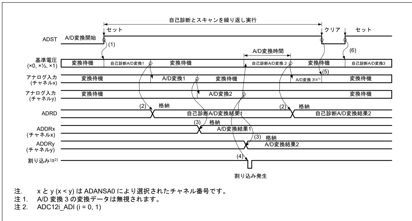
図 42.20 連続スキャンモードの基本動作例 (アナログ入力 (チャンネル x、y) 選択+自己診断)
