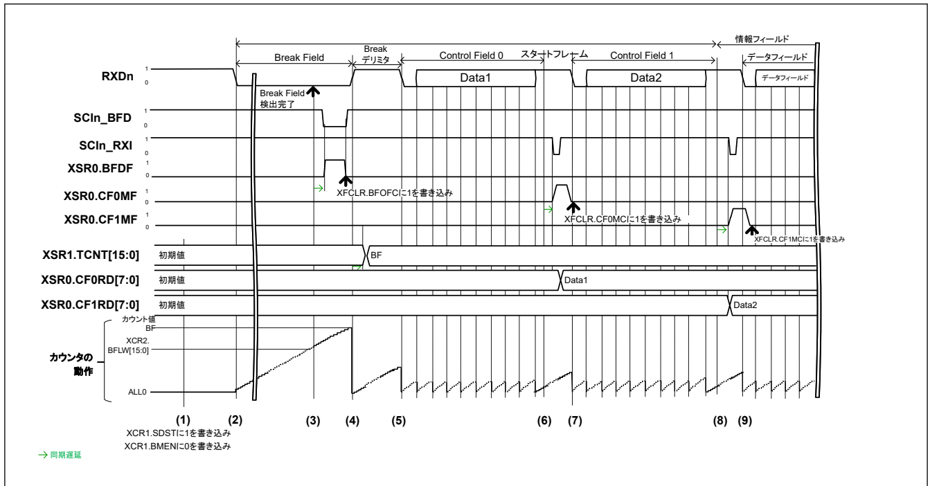
図 30.105 スタートフレームの通常受信例 (PIB は未使用)
