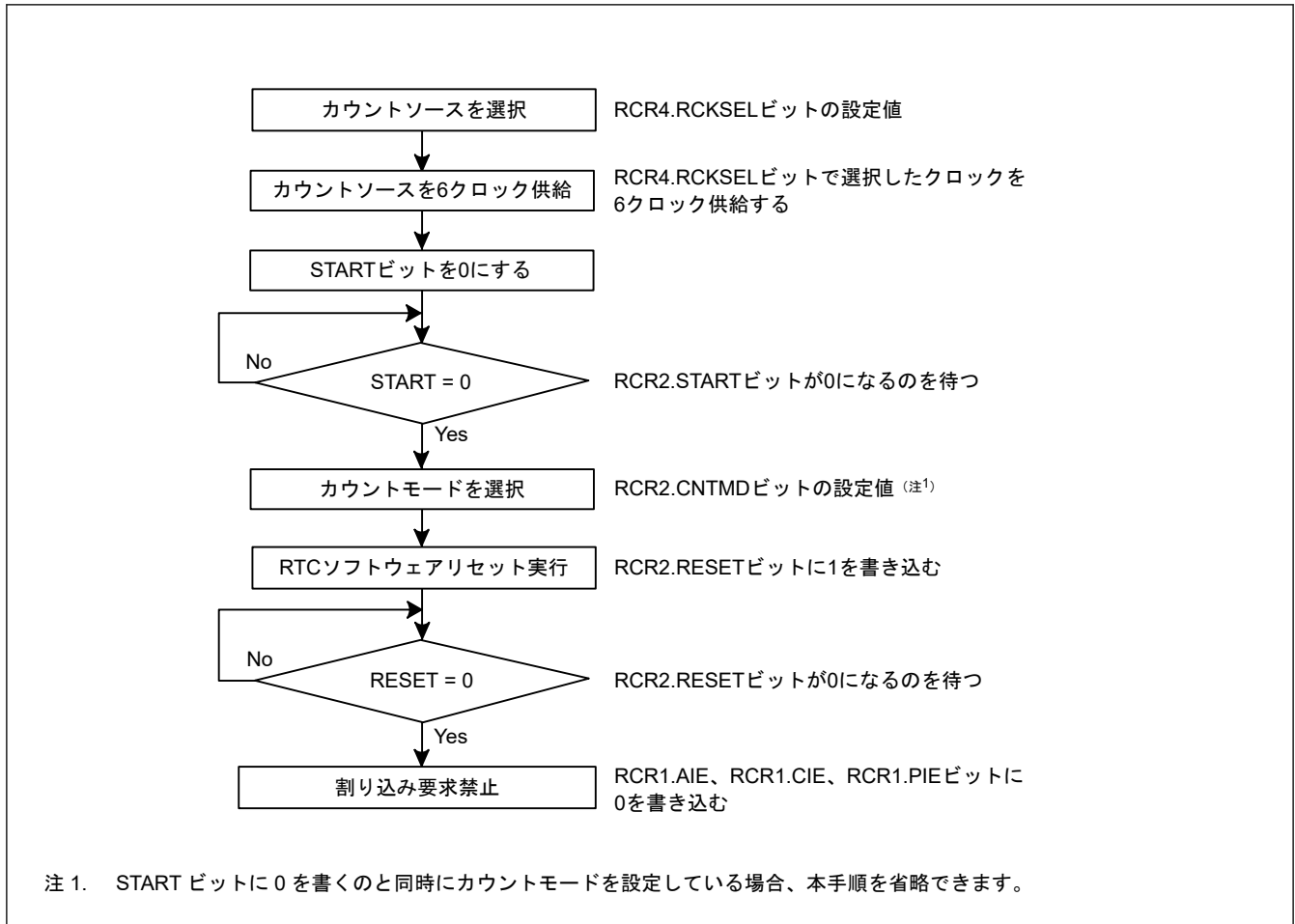
図 24.14 RTC を使用しない場合の初期化手順
