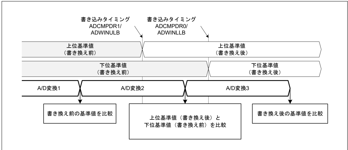
図 42.5 書き換え前後の上側基準値と下側基準値の比較
