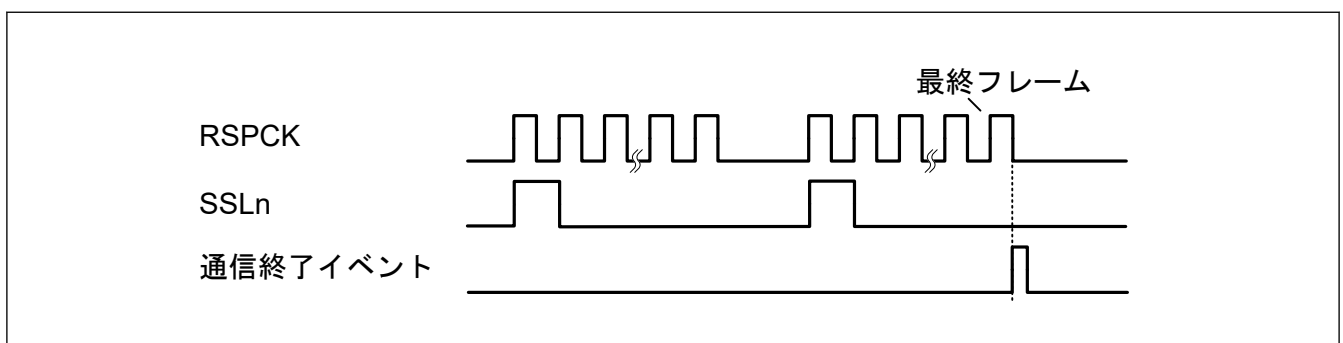
図 34.84 通信終了イベント出カタイミング (受信専用スレーブモード、TI-SSP 動作)
