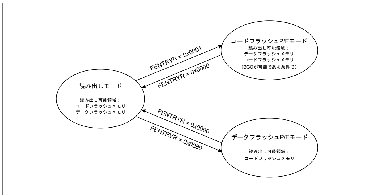
図 49.7 フラッシュシーケンサのモード
