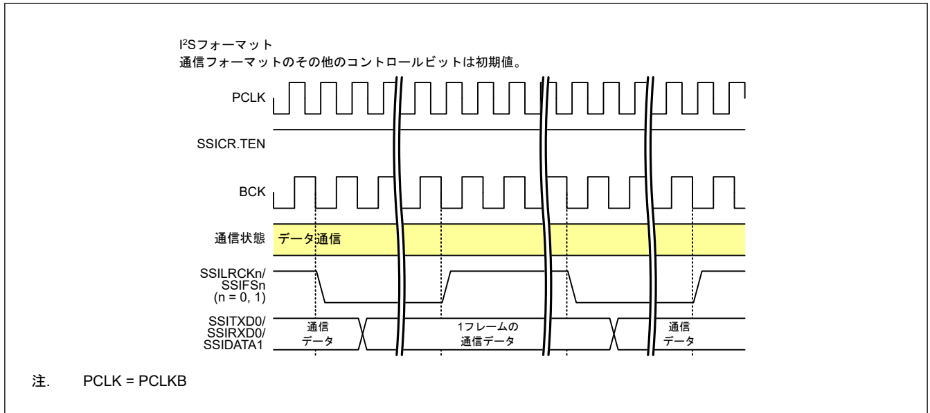
図 37.47 データ通信の継続
