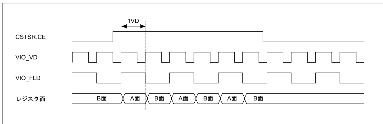
図 50.31 RVS = 1 のときのレジスタ面切り替えタイミング
