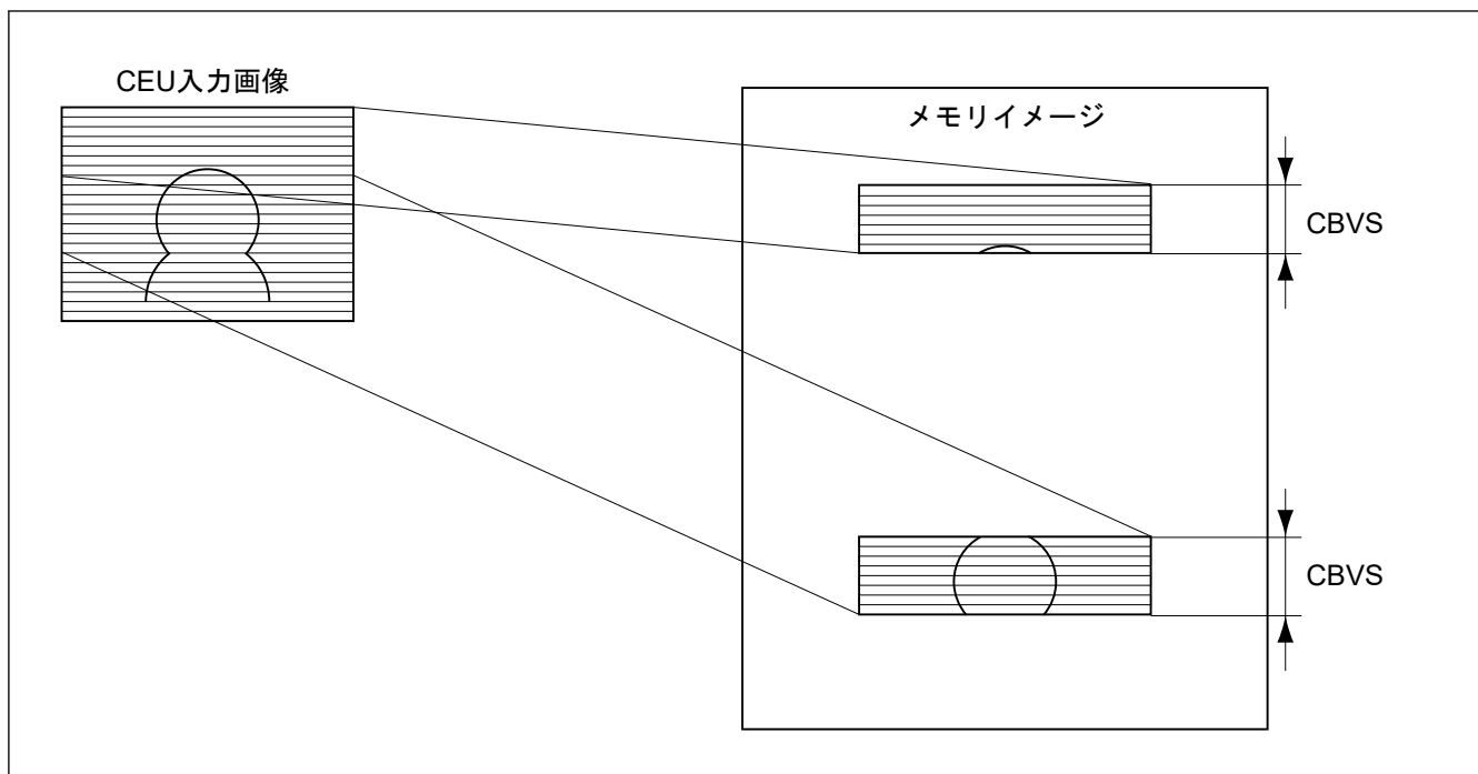
図 50.40 バンドル書き込みキャプチャ画像のメモリ格納イメージ
