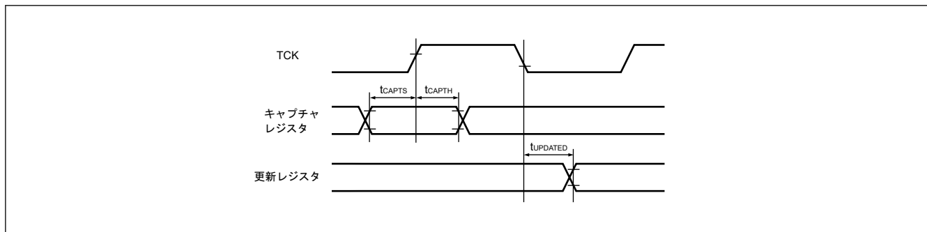
図 52.88 バウンダリスキャン入出力タイミング (2)
