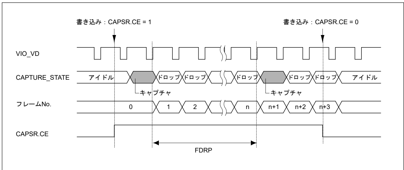
図 50.9 FDRP ビットの設定値とフレームドロップタイミング
