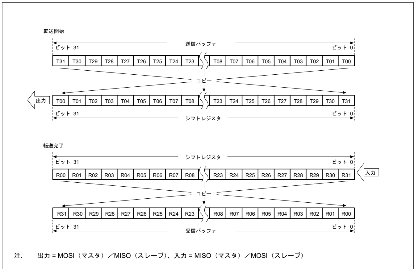
図 34.17 LSB ファースト転送 (32 ビットデータ/パリティ機能無効)
