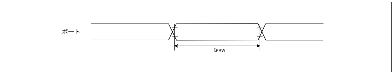
図 52.27 I/O ポート入力タイミング
