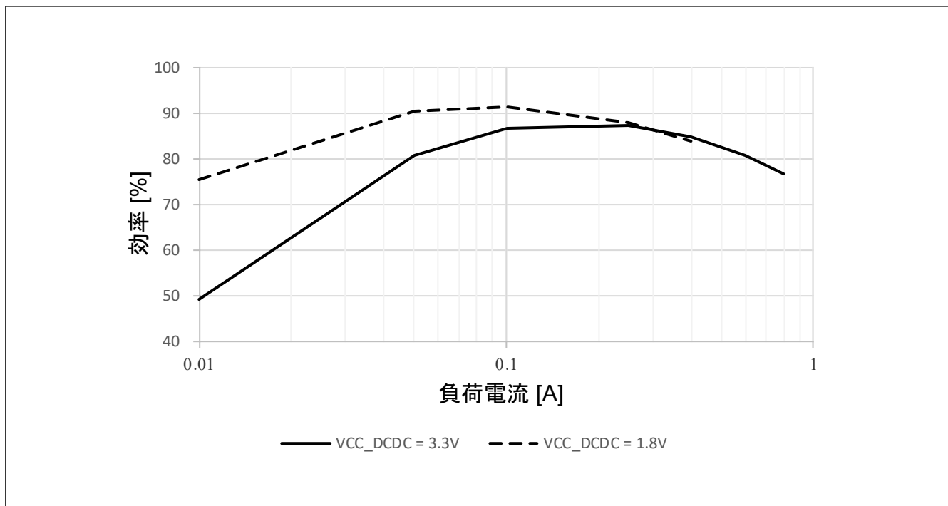
図 52.9 High-speed モード、 T_j = 25^\circ\text{C} における標準 DCDC 効率 (%) と負荷電流 (A)
