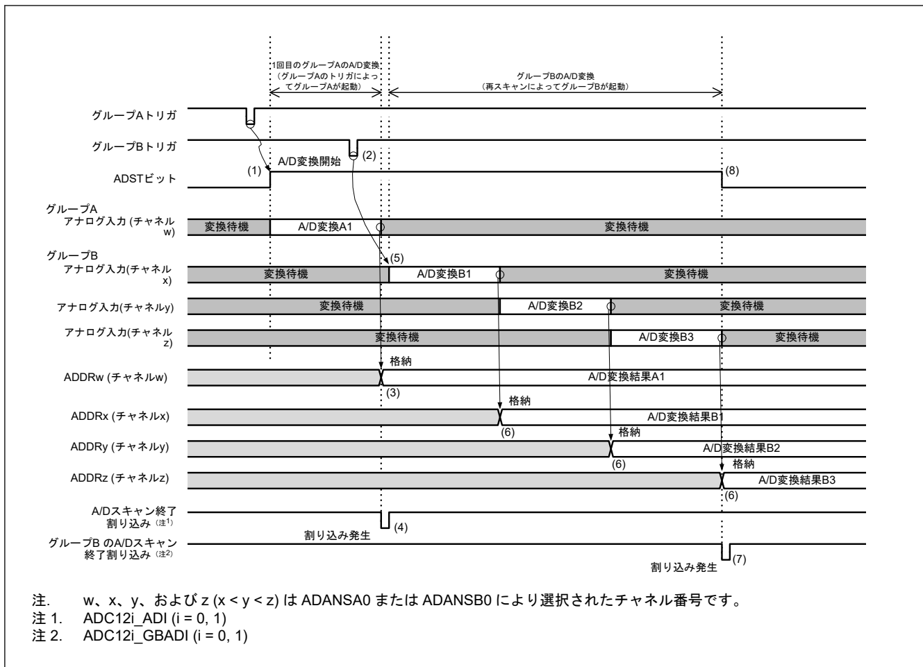
図 42.29 グループ優先動作の例 1-3 : グループ A スキャン中のグループ B トリガ入力、再スキャンあり (ADGSPCR.GBRSCN = 1、ADGSPCR.GBRP = 0、および ADGSPCR.LGRRS = 0 の場合)
