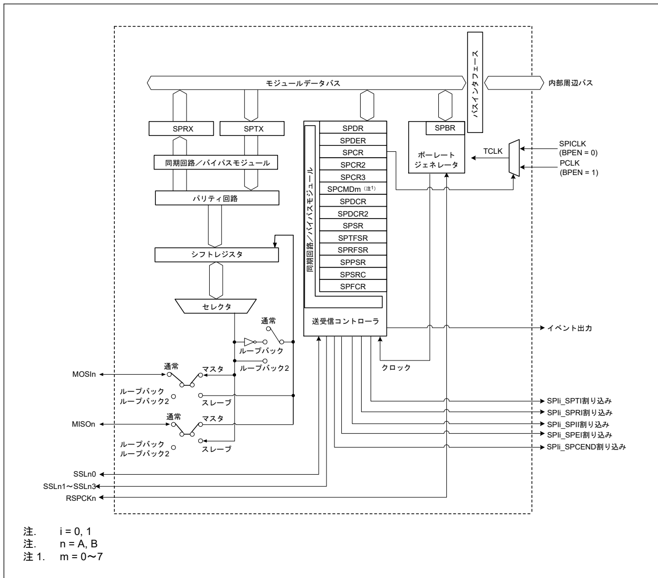
図 34.1 SPIのブロック図
