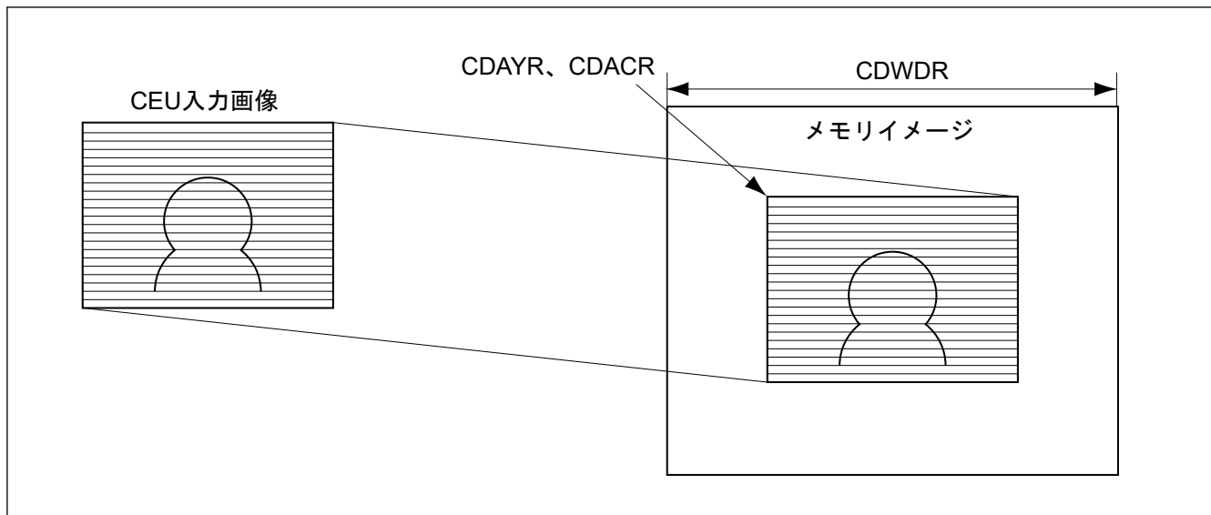
図 50.24 フレームキャプチャ画像および片フィールドキャプチャ画像のメモリ格納イメージ
