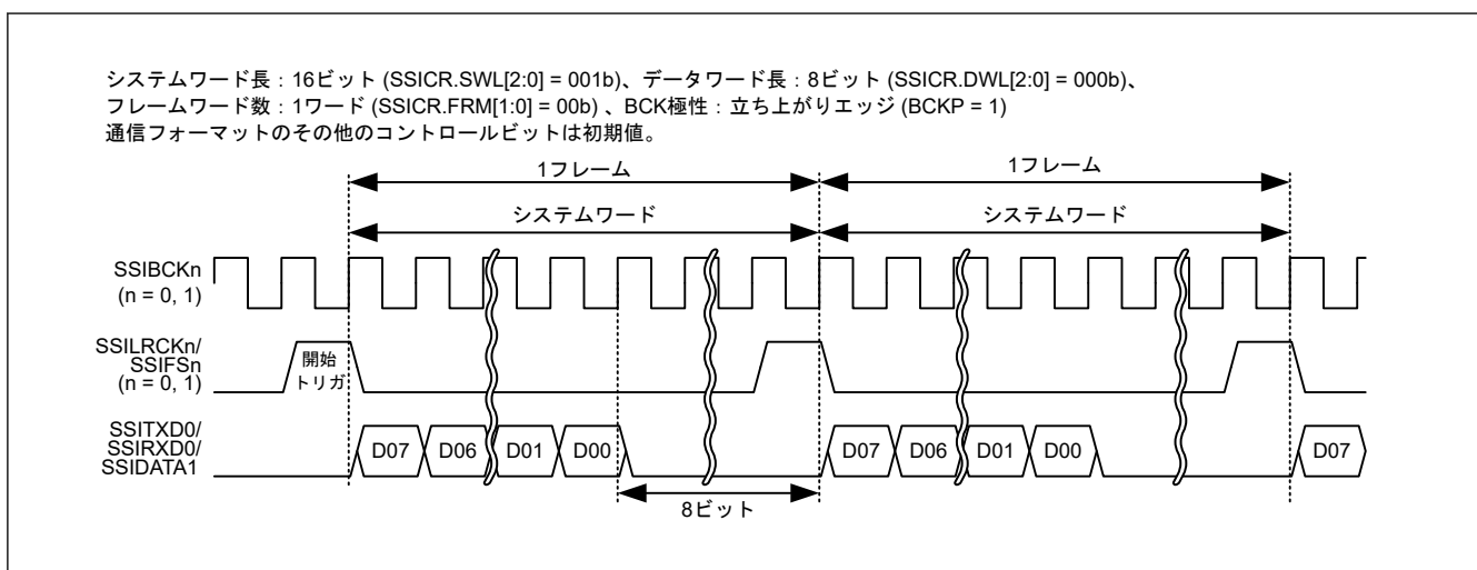
図 37.39 モノラルフォーマットにおけるショートフレーム（パディングあり、システムワード長 > データワード長）
