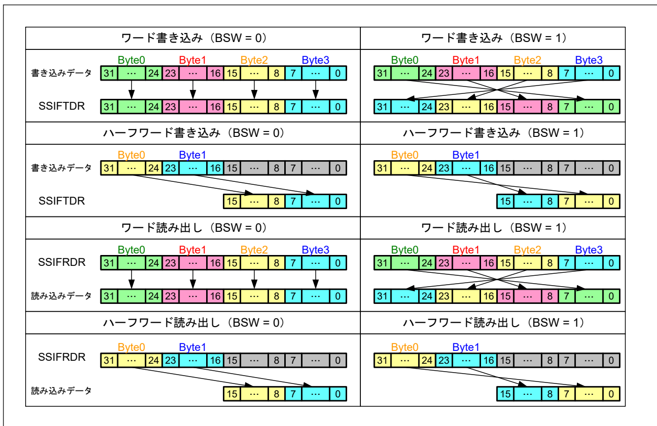
図 37.24 バイトスワップの動作例
