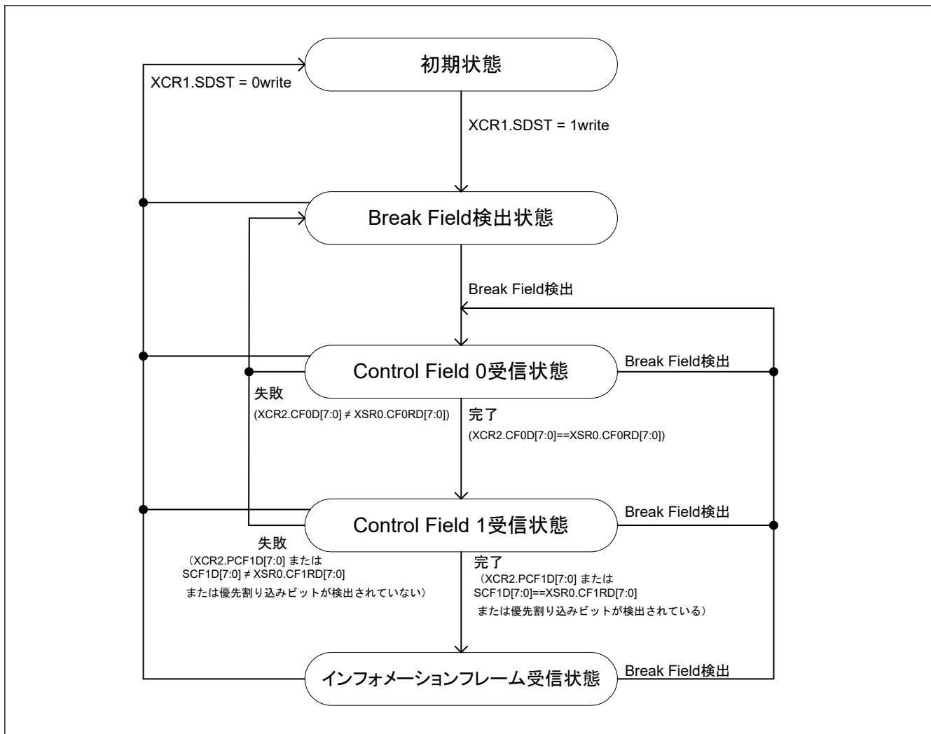
図 30.108 スタートフレーム受信の状態遷移図
