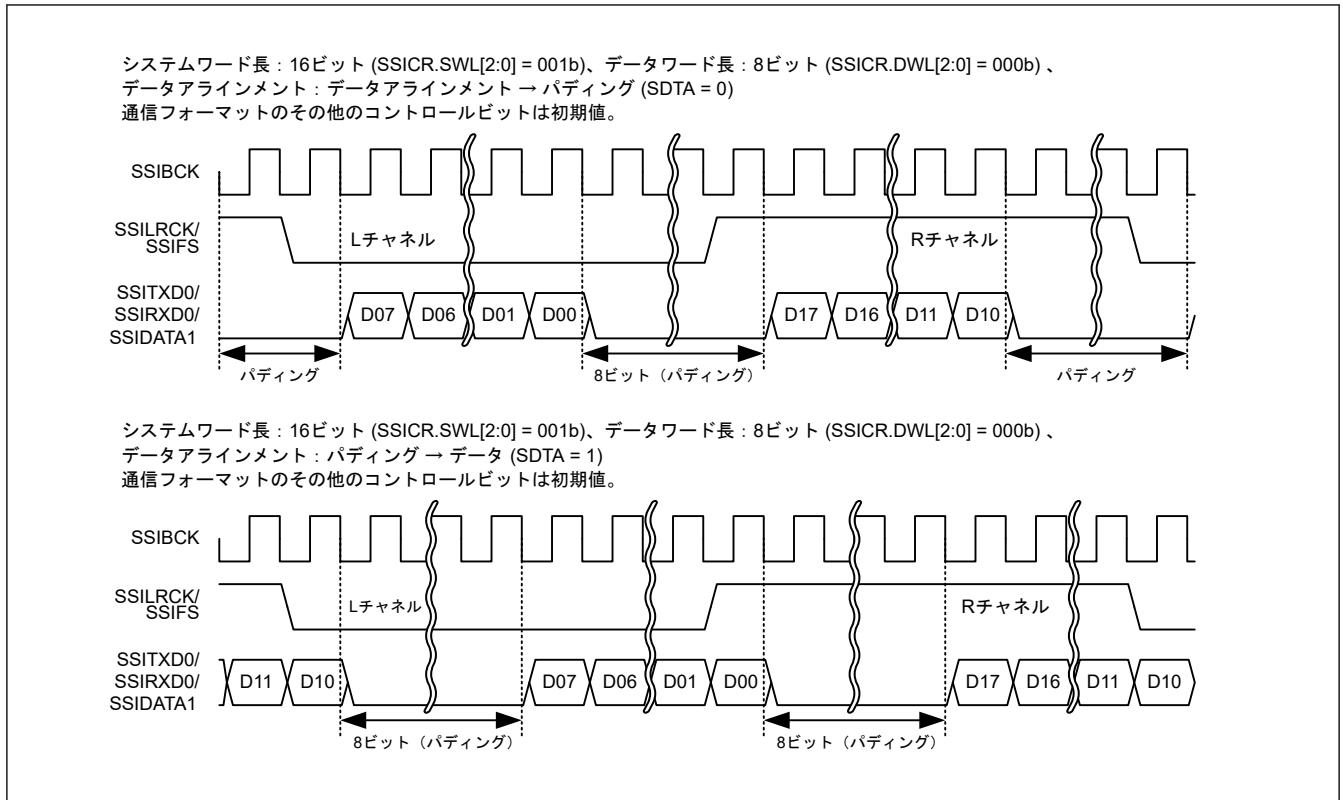
図 37.10 パディングビットを伴うシリアルデータのアライメント設定
