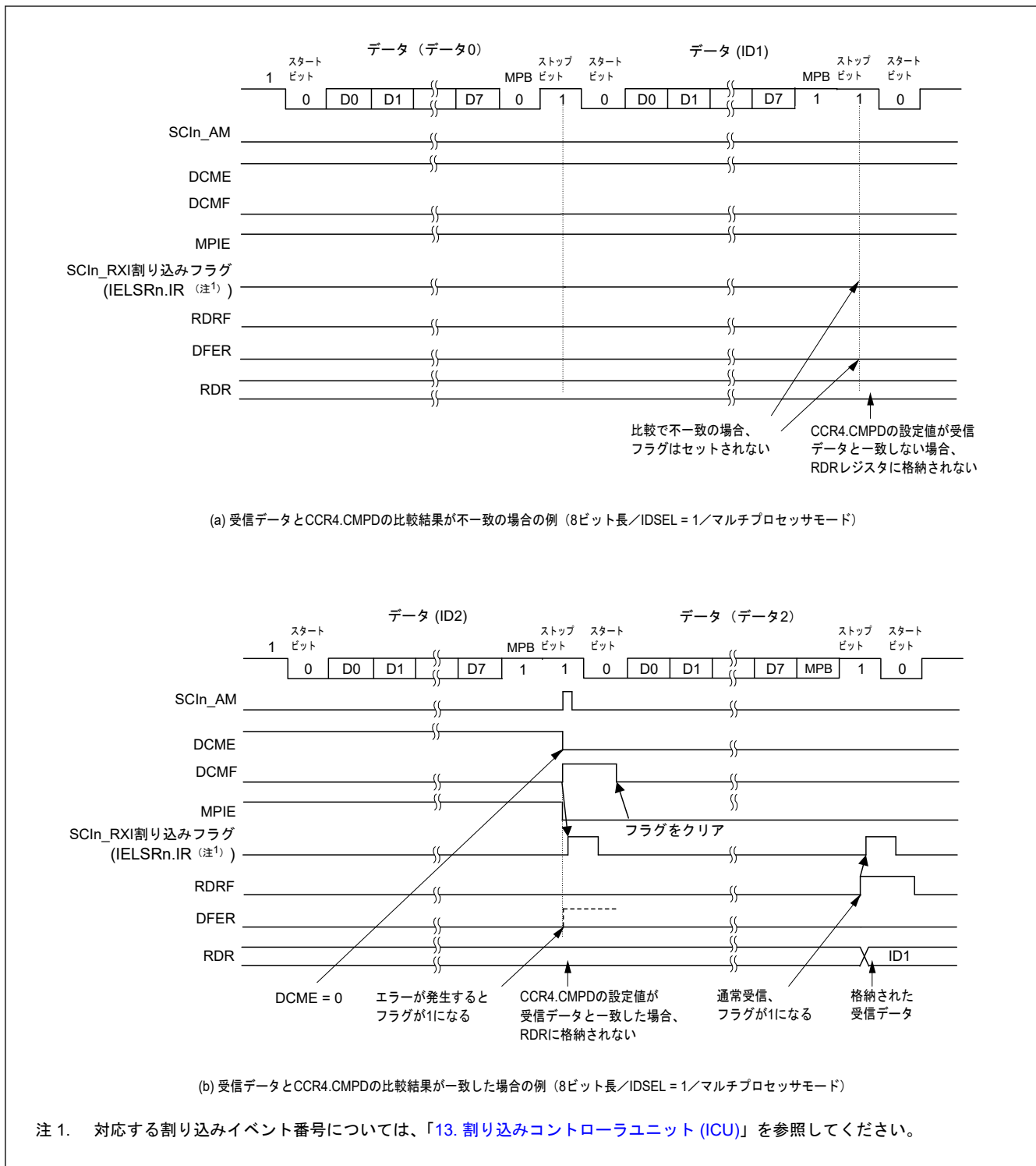
図 30.10 アドレス一致検出の例 (2) (マルチプロセッサモード)
