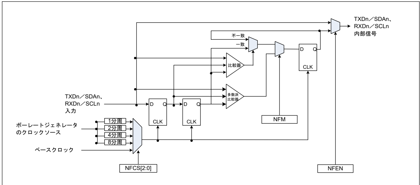
図 30.113 デジタルノイズフィルタ回路のブロック図
