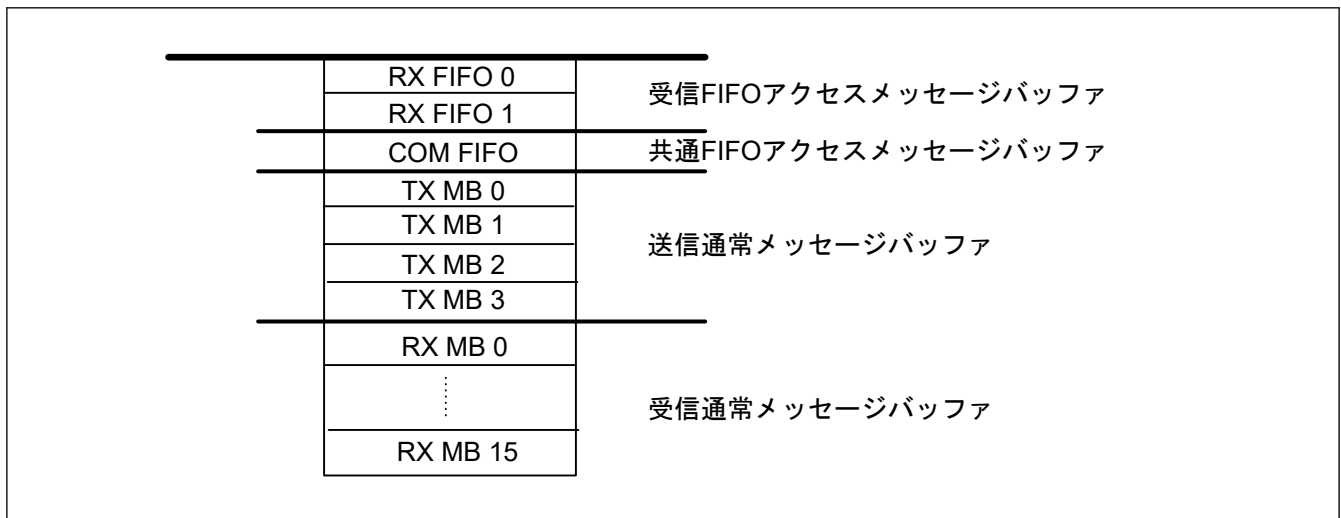
図 32.28 メッセージバッファの構成
