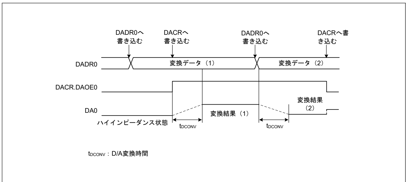
図 43.2 DAC12 の動作例
