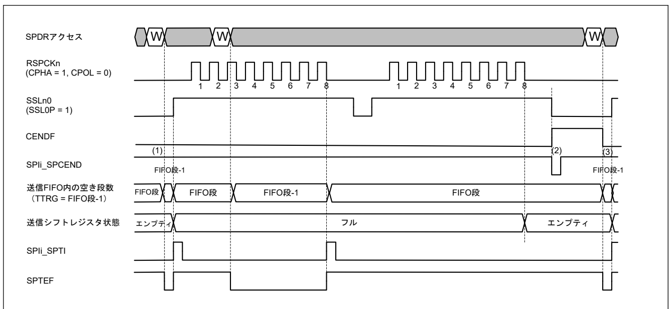
図 34.40 通信終了割り込み動作例 (SPI 動作/Motorola-SPI 時の送受信/送信スレーブモード)
