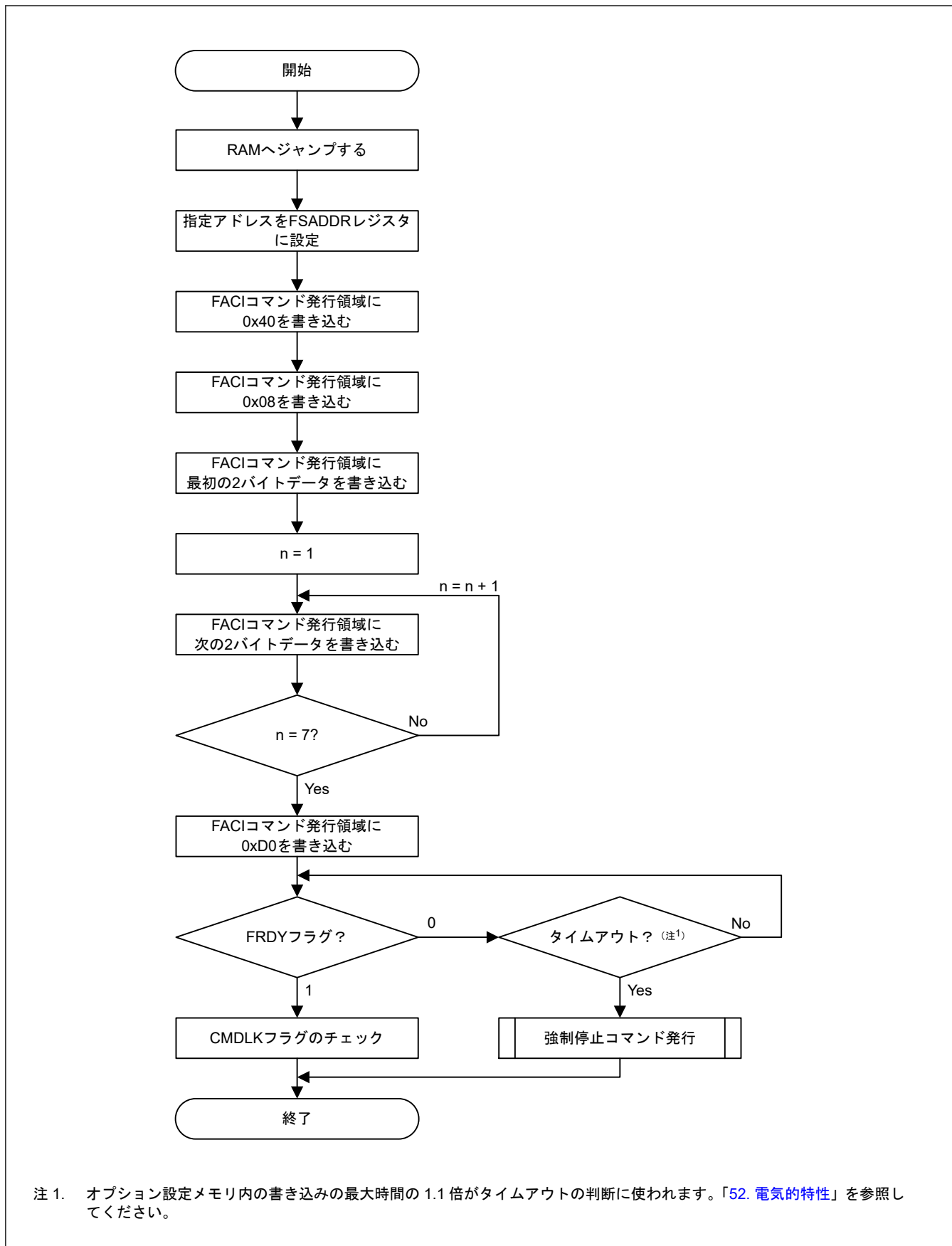
図 49.25 コンフィグレーション設定コマンドの使用フロー
