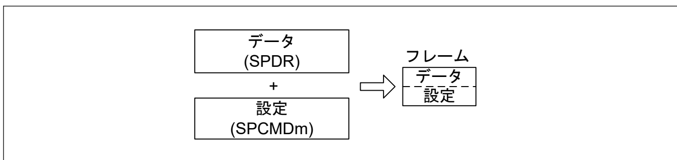
図 34.55 フレームの概念図
