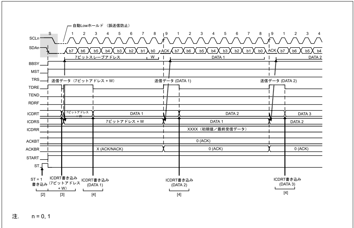
図 31.7 マスタ送信の動作タイミング (1) (7ビットアドレスフォーマット)
