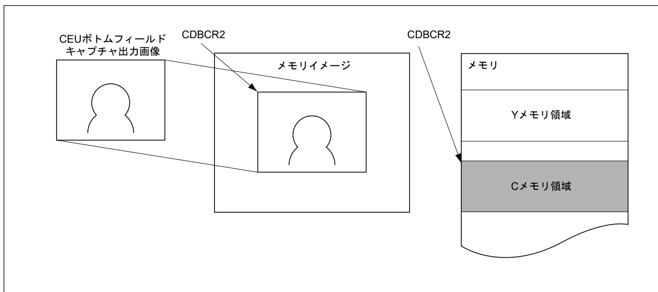
図 50.54 ボトムフィールドキャプチャ画像と色差成分メモリ領域の関係
