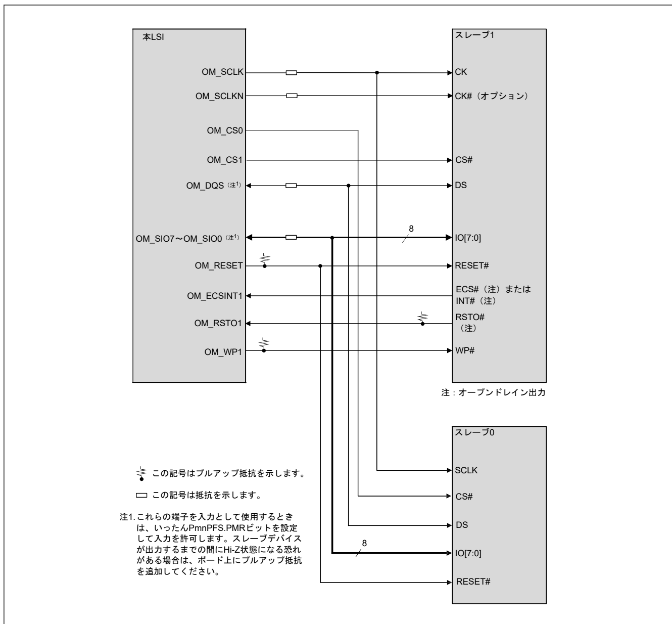
図 35.2 OSPI とメモリデバイス間の接続の例
