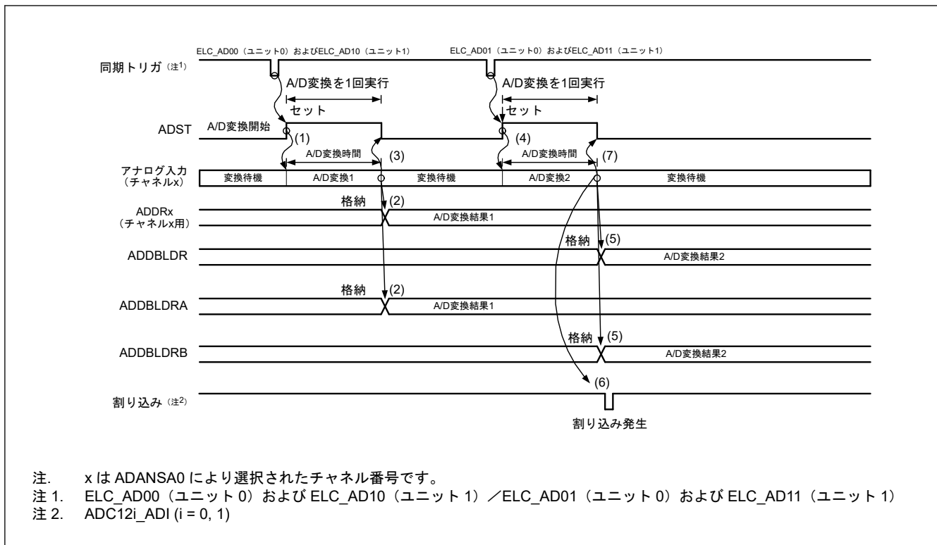
図 42.16 ダブルトリガモードの拡張動作例 (アナログ入力 (チャンネルx) と ELC_AD00 (ユニット0) および ELC_AD10 (ユニット1) / ELC_AD01 (ユニット0) および ELC_AD11 (ユニット1) の2重化選択)
