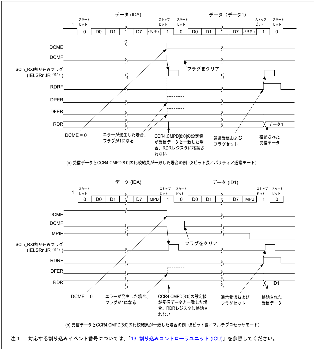
図 30.9 アドレス一致検出の例 (1) (通常モードとマルチプロセッサモード)
