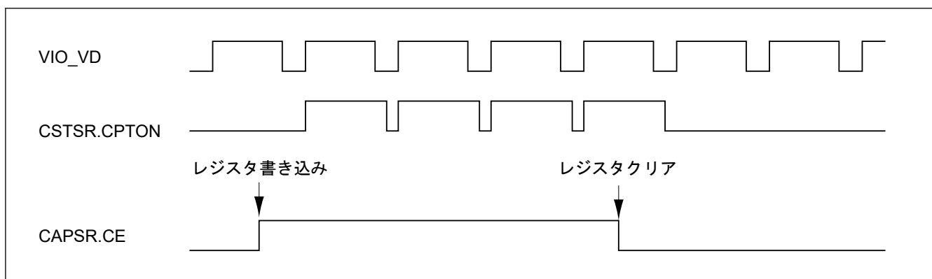
図 50.8 連続フレームキャプチャ
