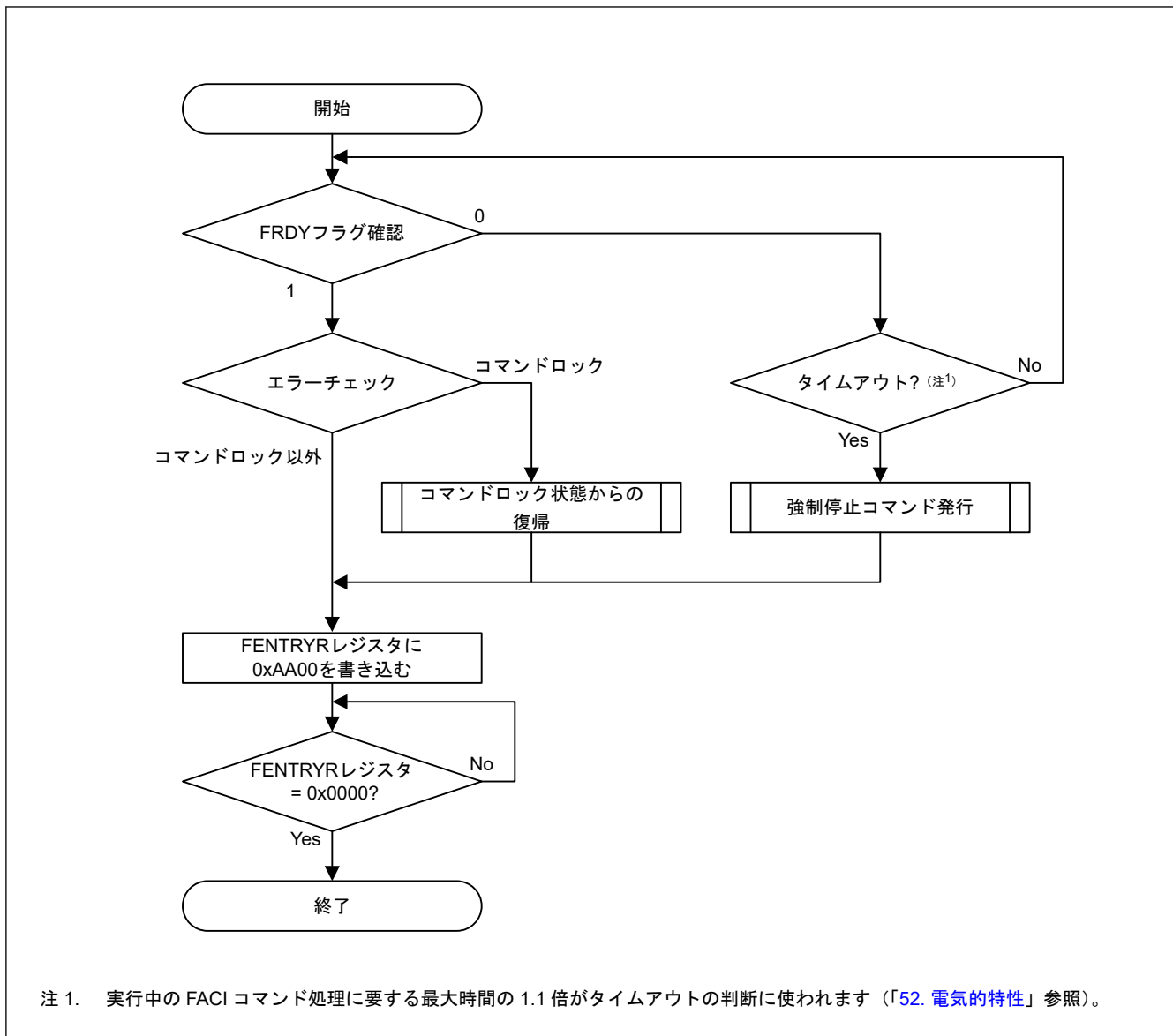
図 49.12 読み出しモードへの遷移手順
