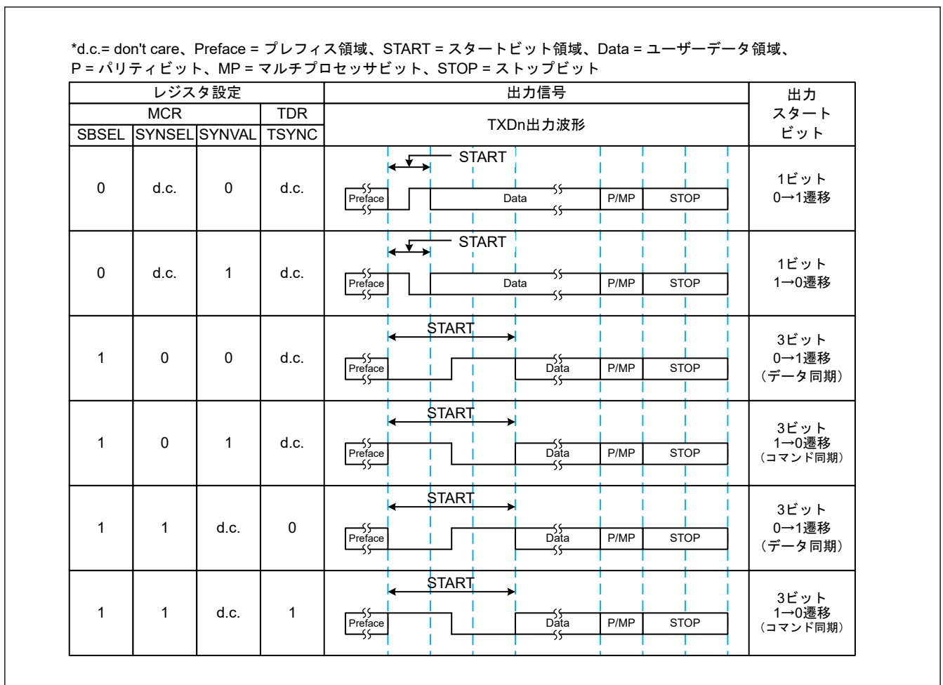
図 30.48 送信時のスタートビット領域に関する設定とフォーマット
