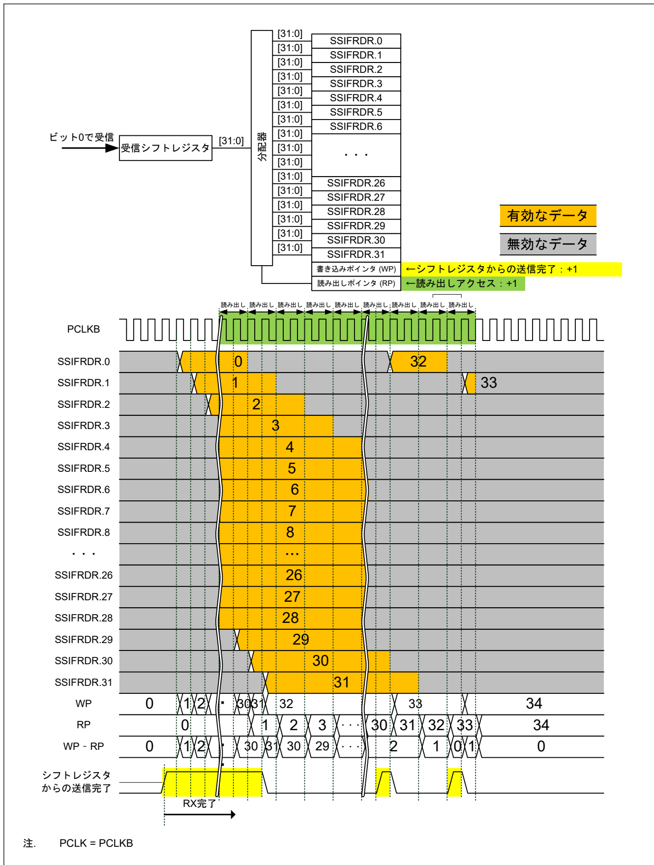
図 37.32 受信 FIFO データレジスタと受信シフトレジスタの構成、および FIFO の動作例
