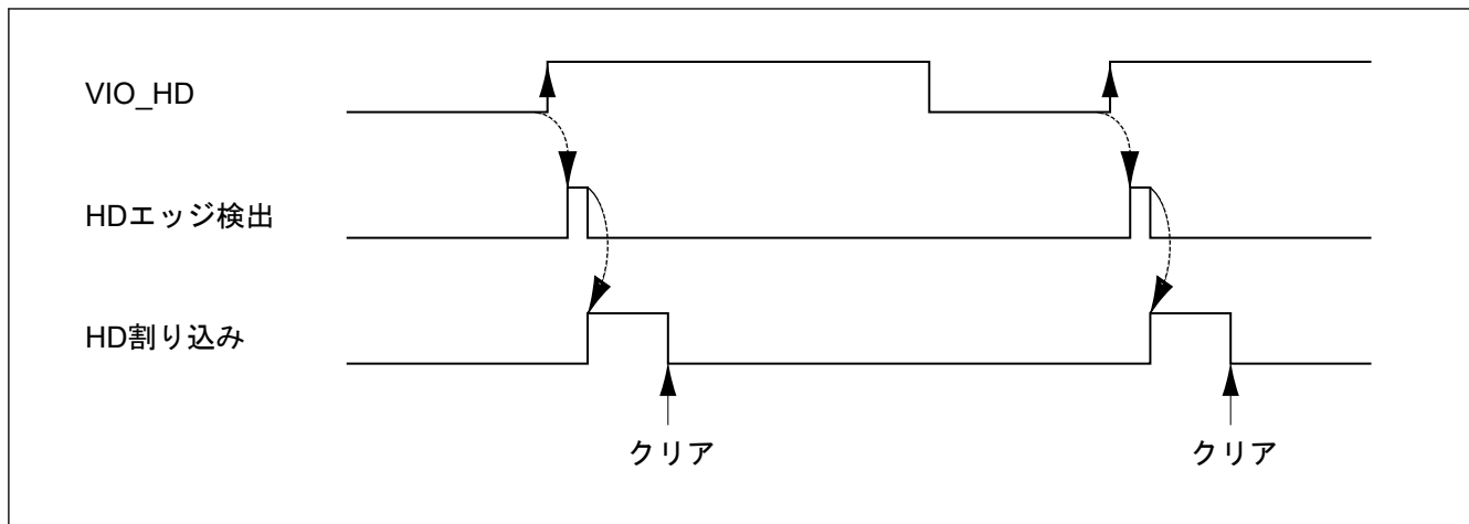
図 50.16 HD が正極性の場合の VIO_HD と HD 割り込みの関係
