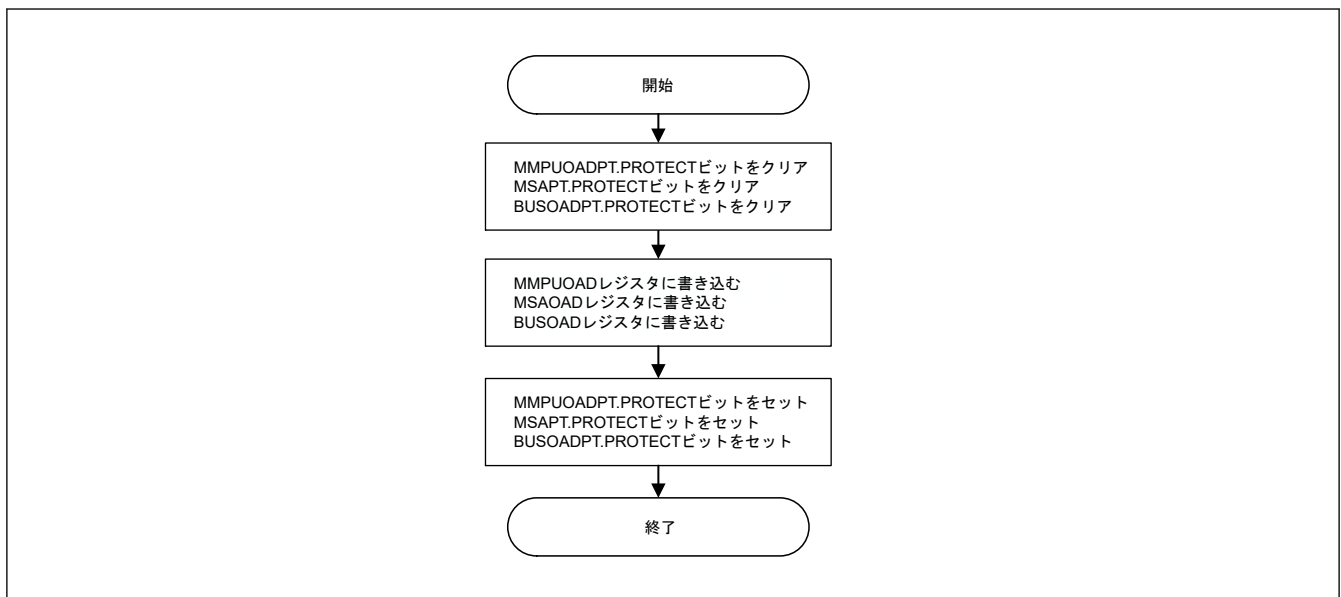
図 14.3 リセット後の OAD 設定フロー
