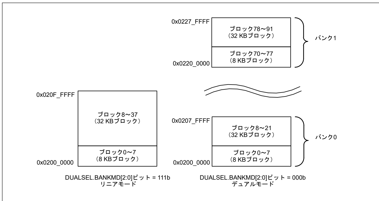
図 49.33 バンクモード切り替えフロー例 (セキュアエアの場合)
