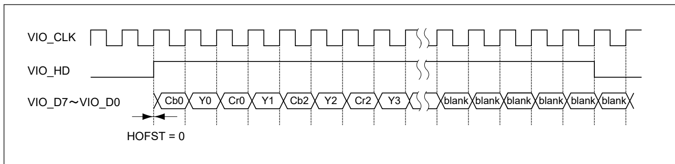
図 50.20 HD がデータイネーブル信号の場合のタイミング
