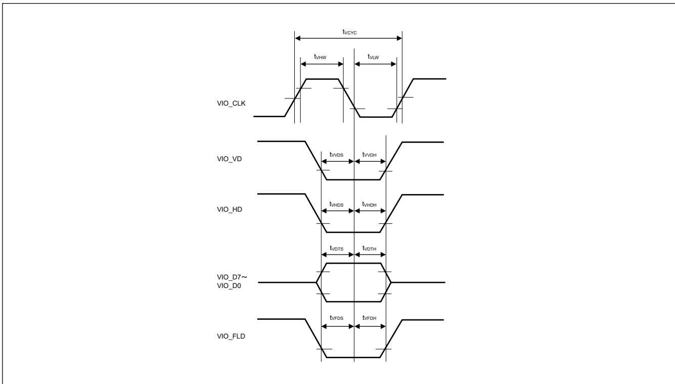
図 52.72 VIO_CLK の立ち下がりエッジによるデータキャプチャのキャプチャエンジンユニットモジュール信号タイミング
