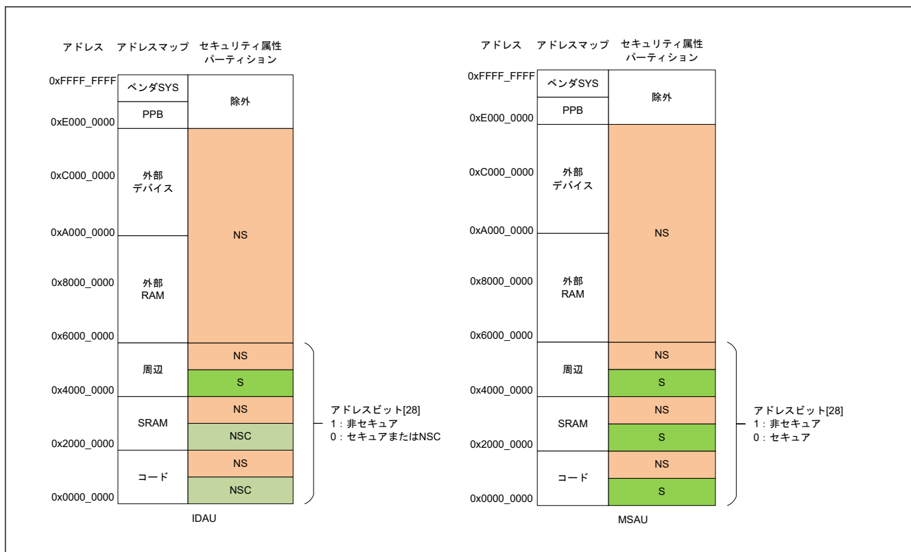
図 40.2 IDAU および MSAU の定義されたセキュリティマップ
