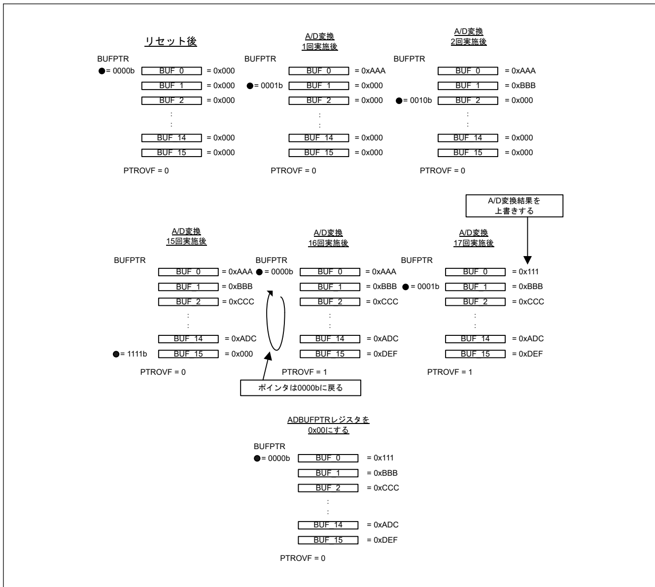
図 42.42 データバッファ、ポインタ、およびオーバーフローフラグの動作概略図
