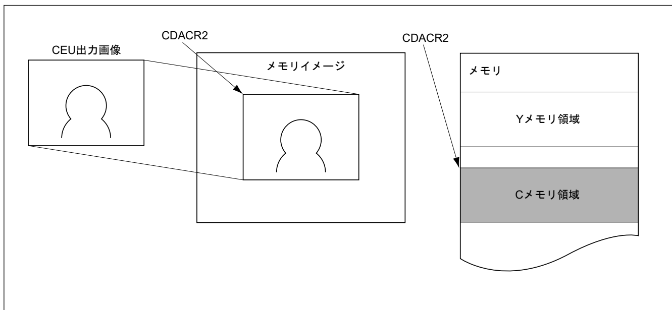
図 50.51 キャプチャ画像と色差成分メモリ領域の関係
