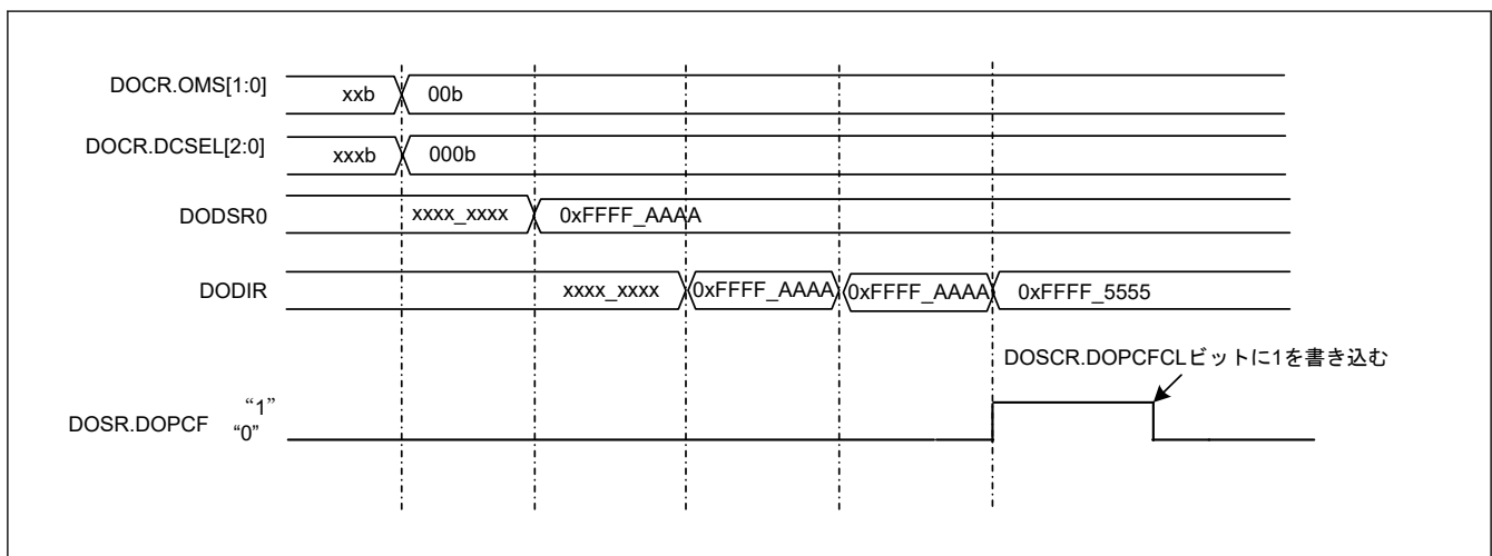
図 46.2 データ比較モードの動作例 (検出条件: 不一致)
