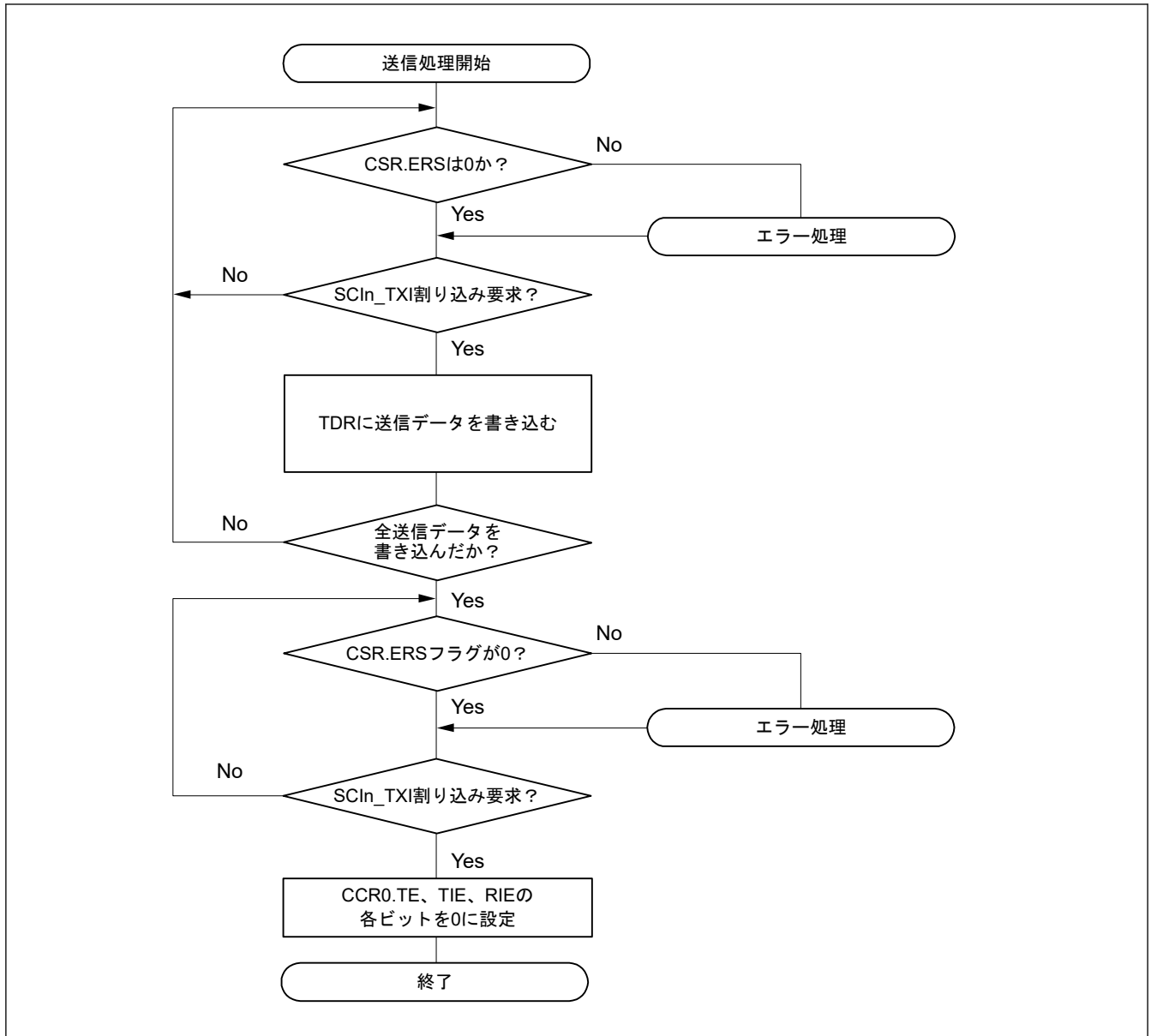
図 30.82 スマートカードインタフェース送信のフローチャート例
