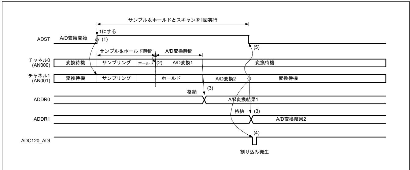
図 42.9 シングルスキャンモードの動作例（チャンネル専用サンプル&ホールド回路使用、AN000 および AN001 選択）
