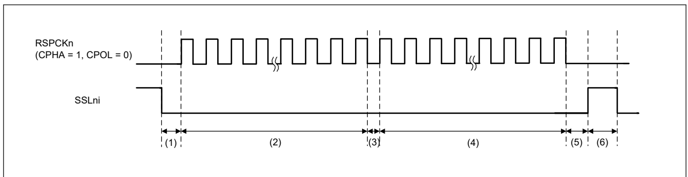
図 34.61 SSLKP ビットを利用したバースト転送の動作例 (BFDS = 1、SPFRF = 0)
