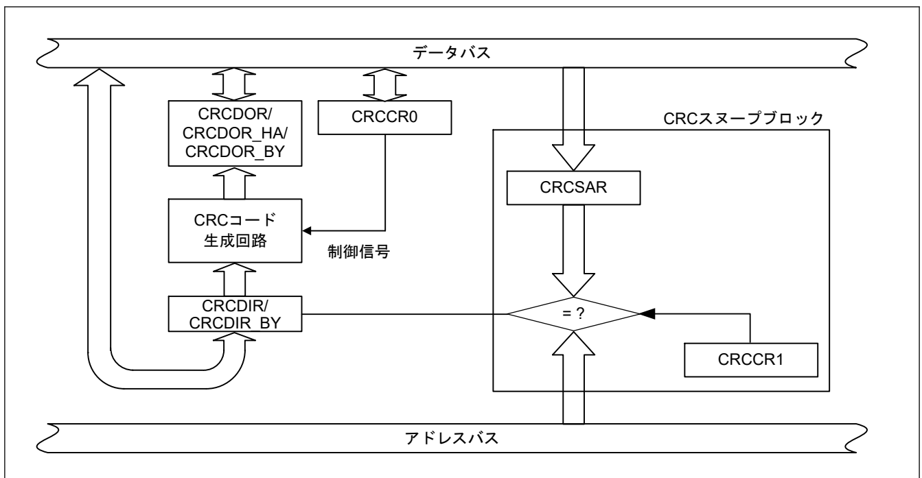
図 38.1 CRC 演算器のブロック図
