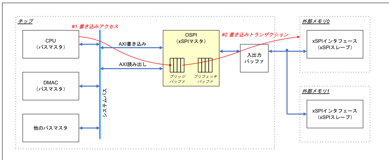
図 35.12 メモリ領域に対する書き込みアクセス
