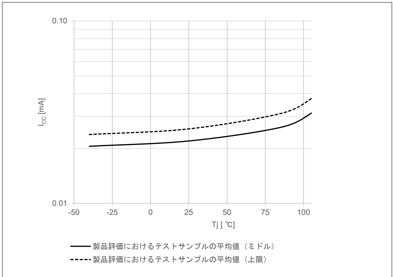
図 52.3 ソフトウェアスタンバイモードにおける温度依存性 ( I_{cc} ) (参考データ)
