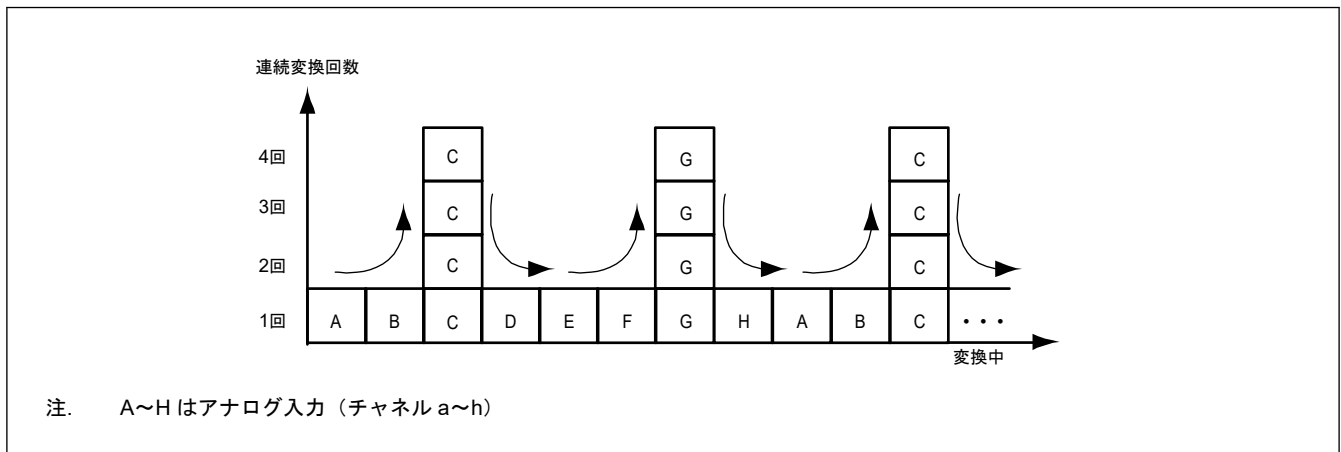
図 42.3 ADADC.ADC[2:0] = 011b および ADADS0 によるアナログ入力 C と G を 1 に選択時のスキャン変換シーケンス
