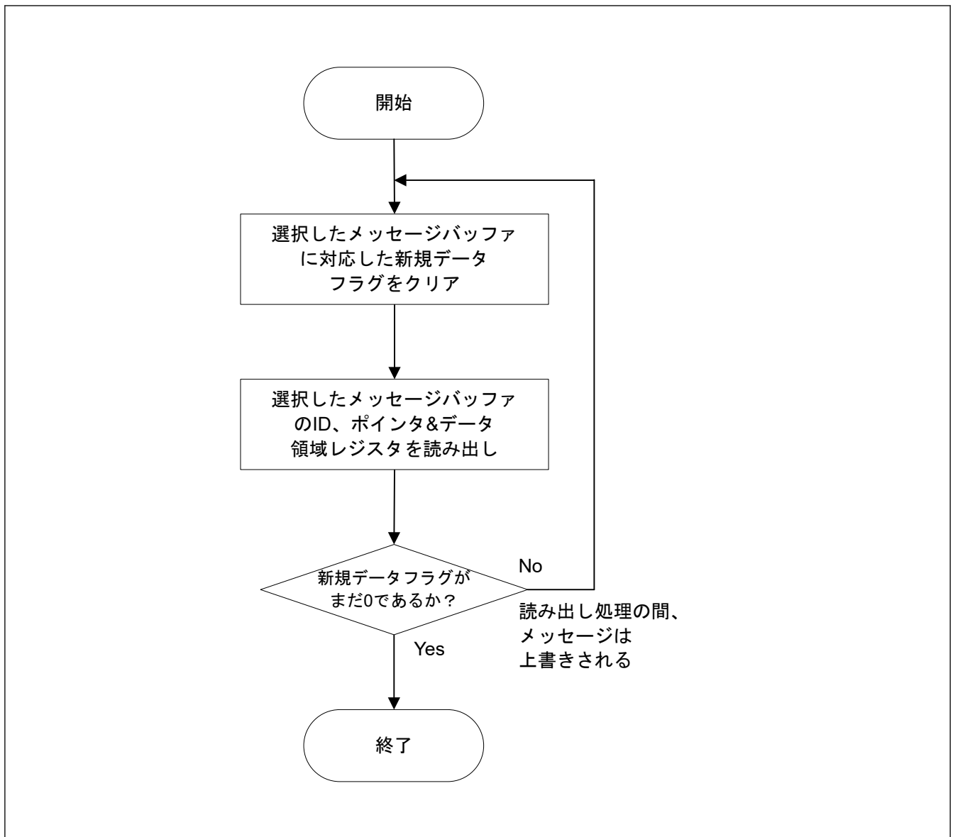
図 32.37 RX メッセージバッファの読み出し手順
