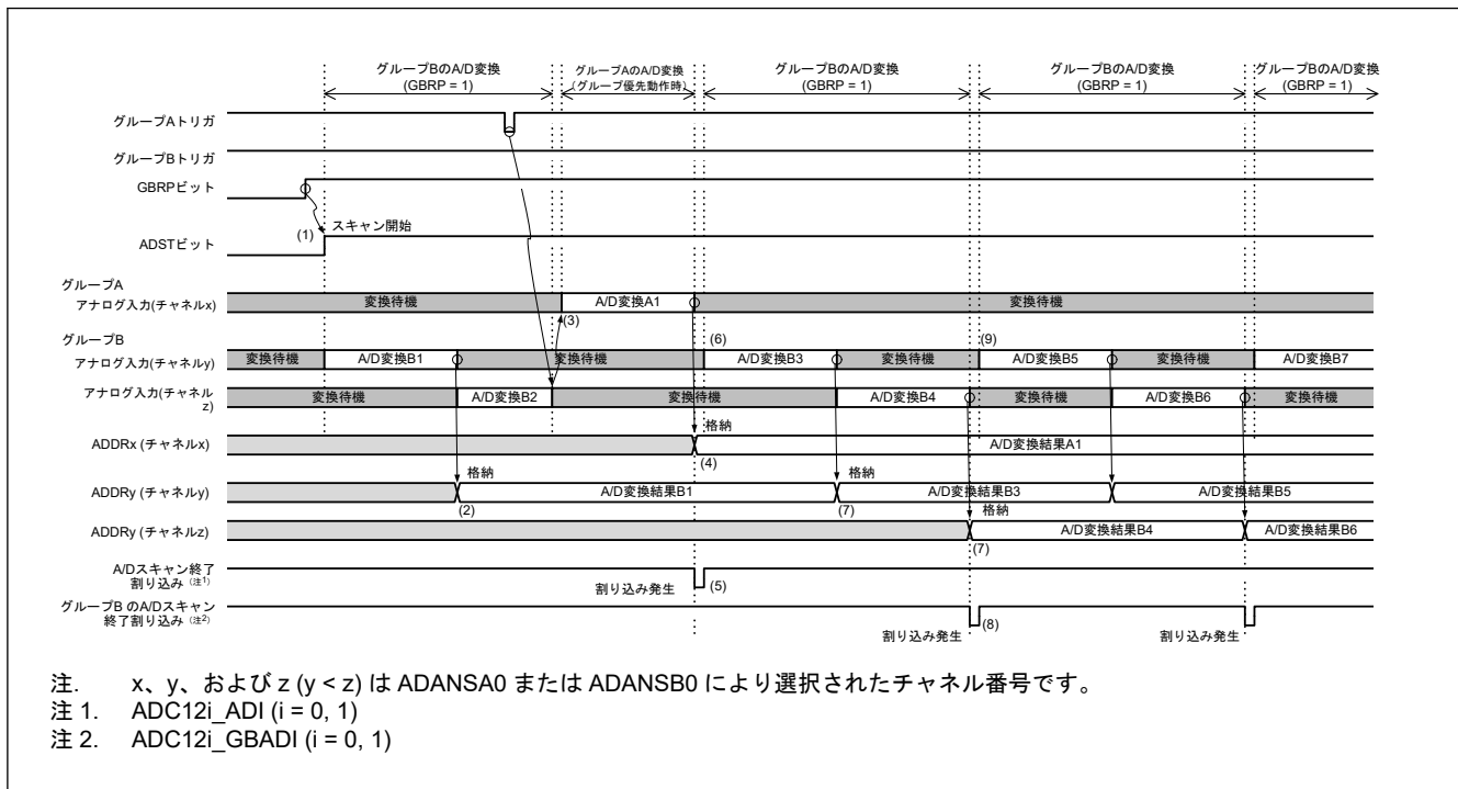
図 42.31 グループ優先動作の例 1-5 : グループ B のシングルスキャン連続動作 (ADGSPCR.GBRP = 1, ADGSPCR.LGRRS = 0 の場合)
