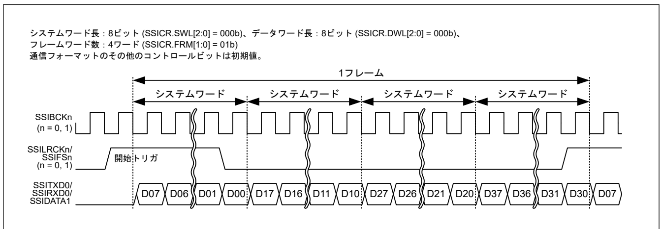
図 37.41 TDM フォーマット (パディングなし、システムワード長 = データワード長)
