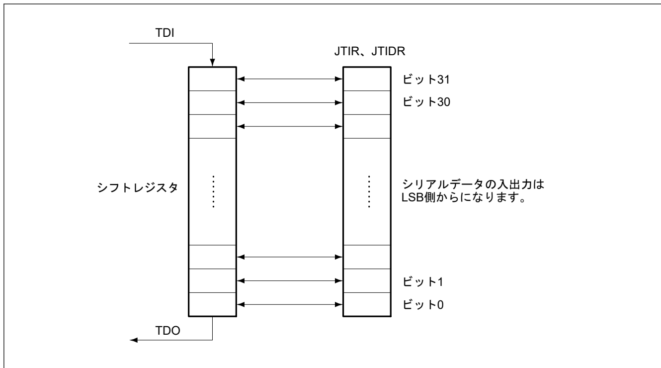
図 39.3 シリアルデータ入出力
