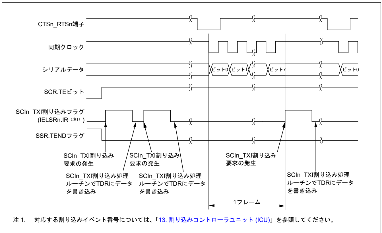
図 30.63 クロック同期式モードにおけるシリアル送信の動作例 (送信開始時に CTS 機能を使用する場合)
