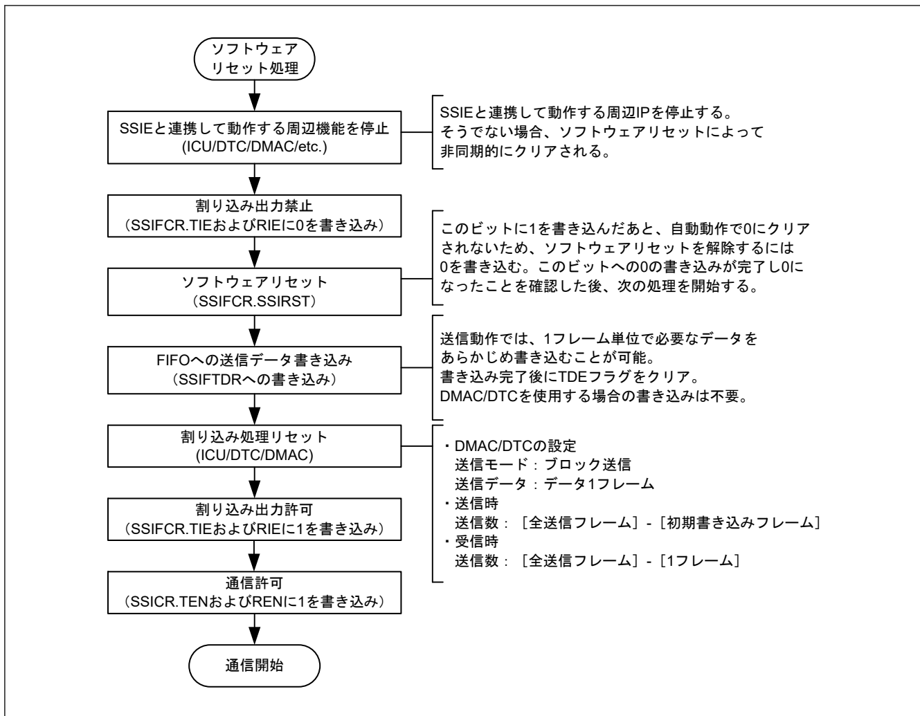
図 37.62 ソフトウェアリセット手順 (CPU 動作手順)
