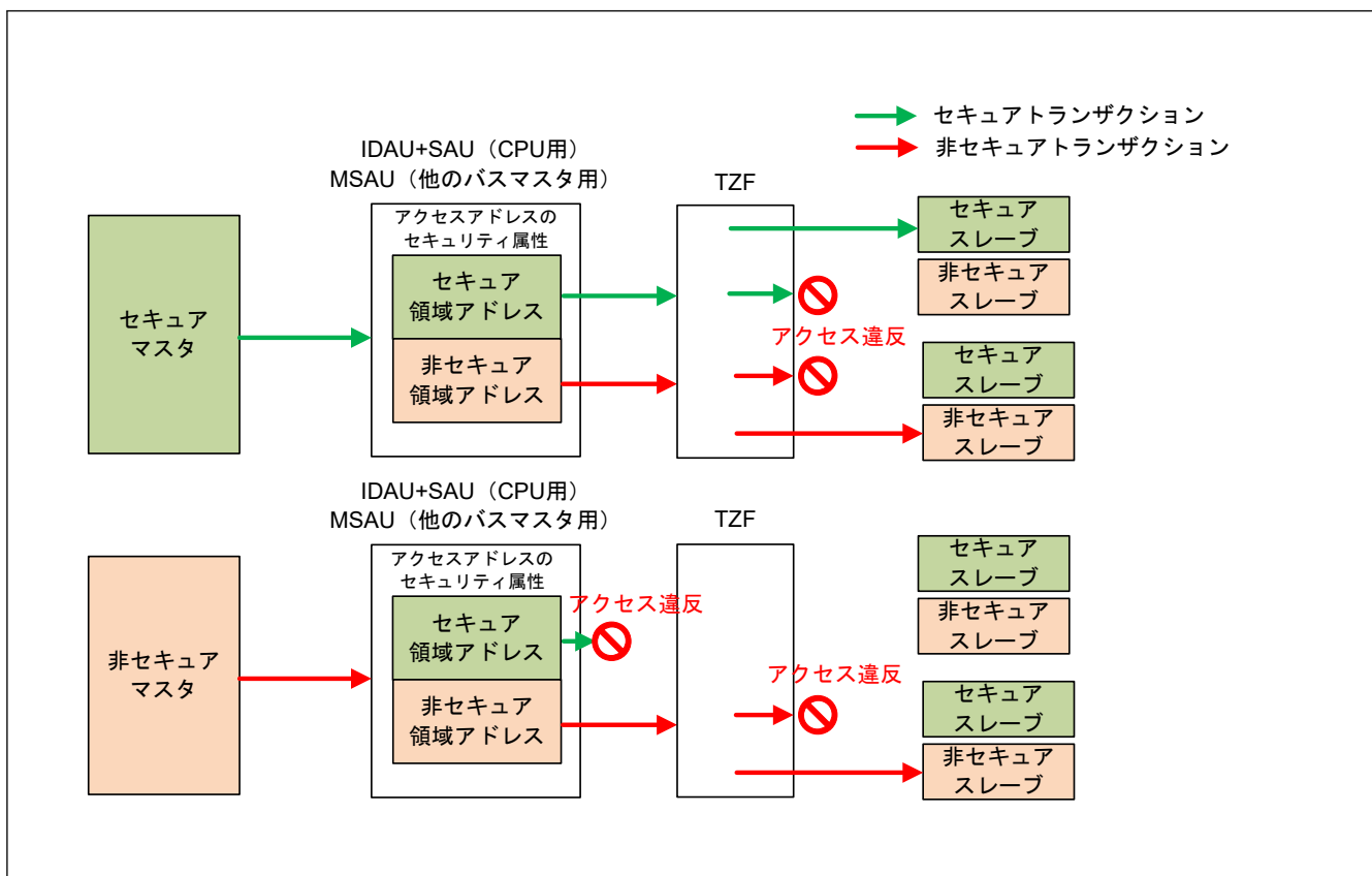
図 40.1 各マスタが発行できるトランザクション
