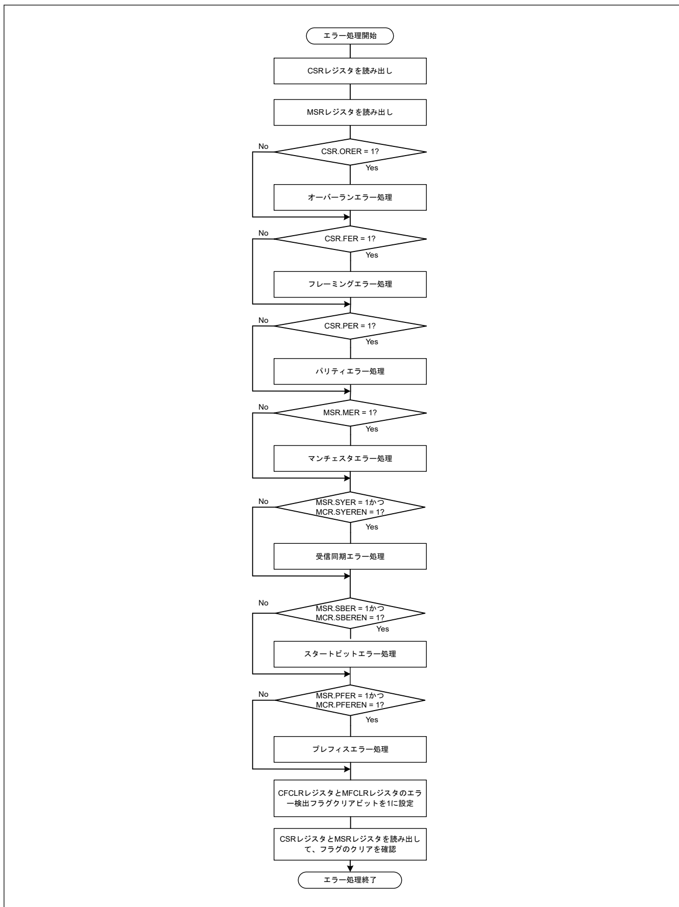
図 30.58 マンチェスタモードにおけるシリアル受信フローチャートの例 (エラー処理)
