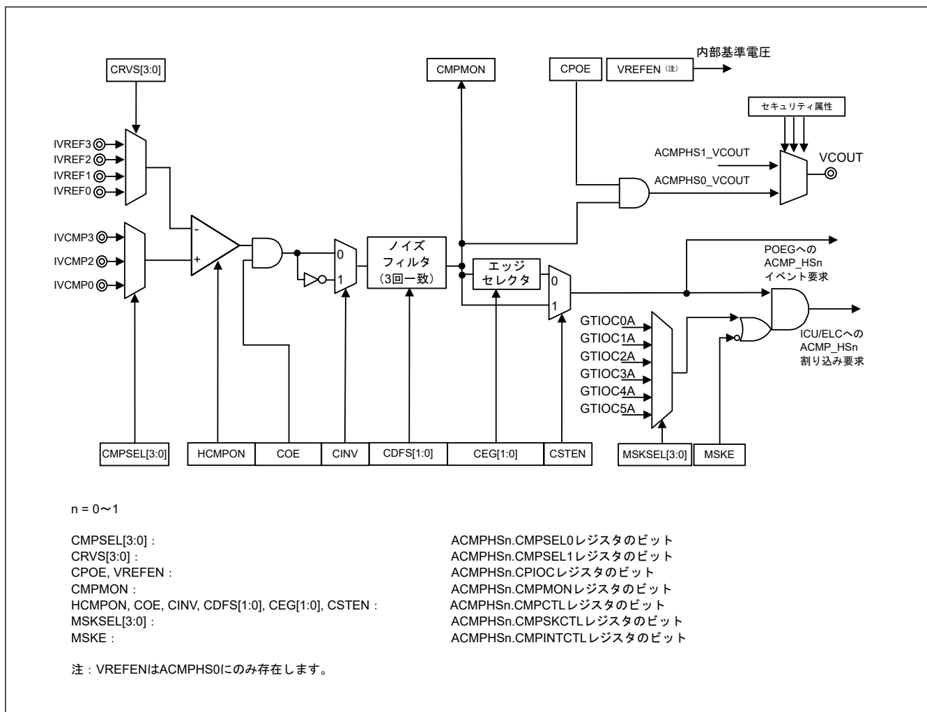
図 45.1 ACMPHS ブロック図
