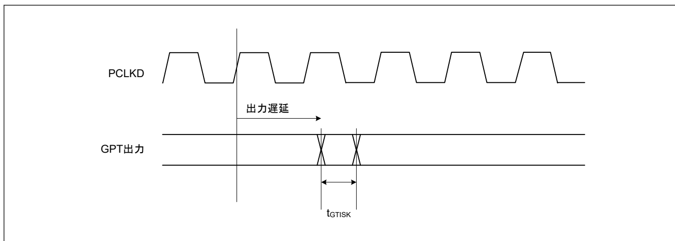
図 52.31 GPT 出力遅延スキュー
