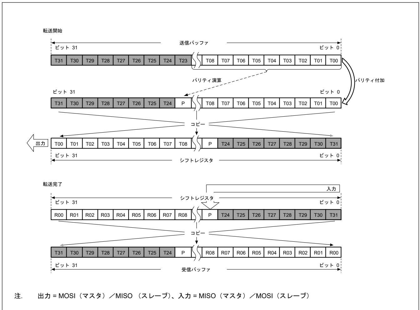
図 34.22 LSB ファースト転送 (24 ビットデータ/パリティ機能有効)
