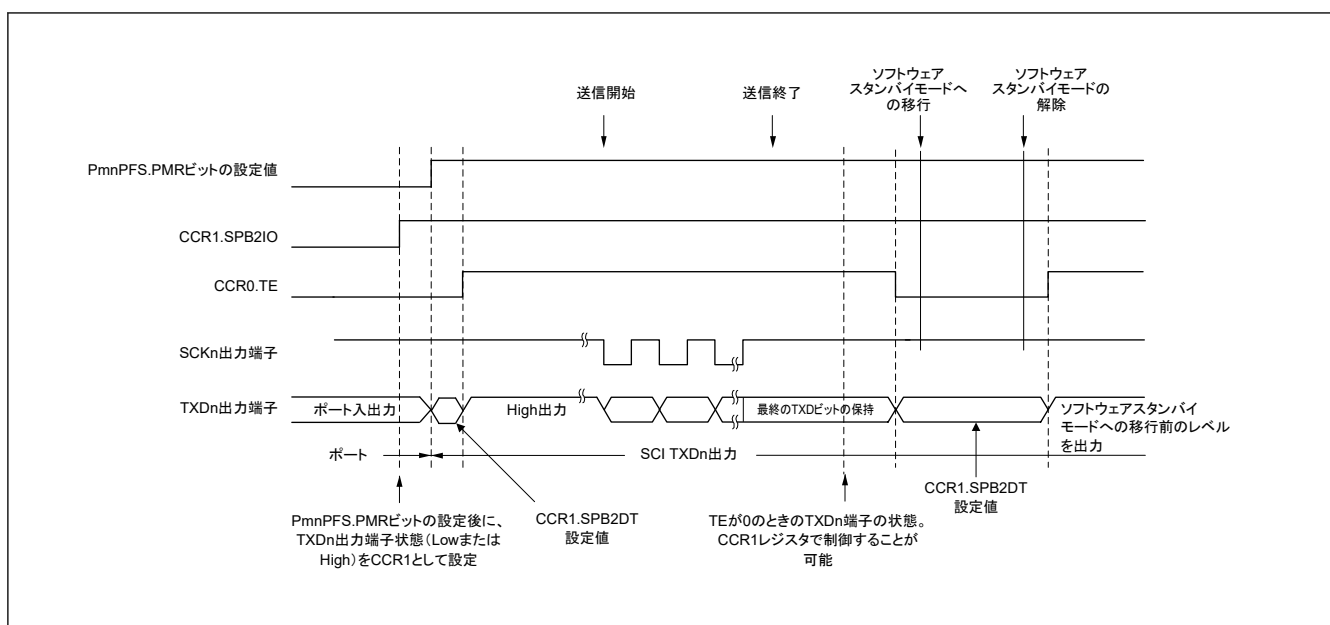
図 30.119 ソフトウェアスタンバイモード遷移時のポートの端子状態 (内部クロック、クロック同期送信)
