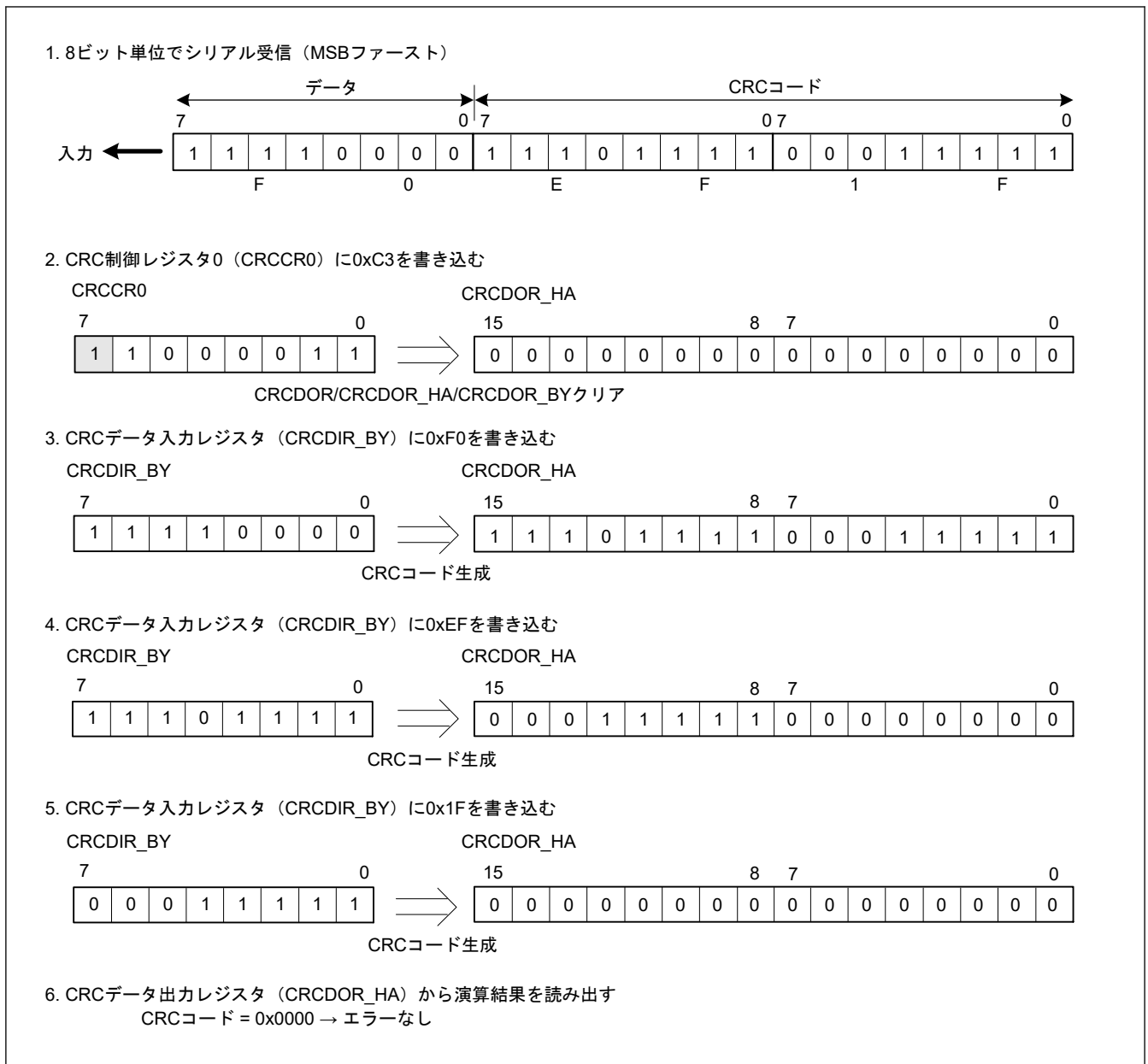
図 38.5 MSBファーストのデータ受信
