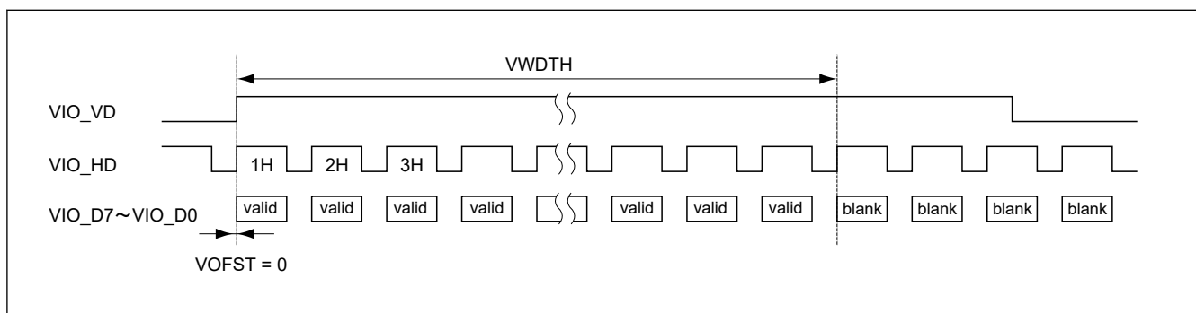
図 50.21 垂直キャプチャタイミング
