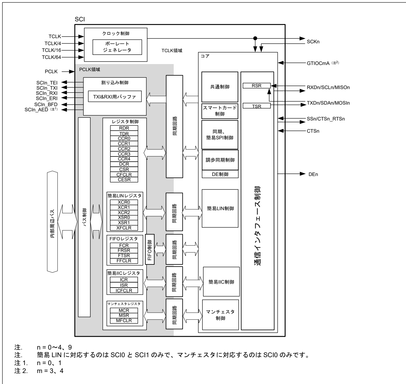
図 30.1 SCIのブロック図
