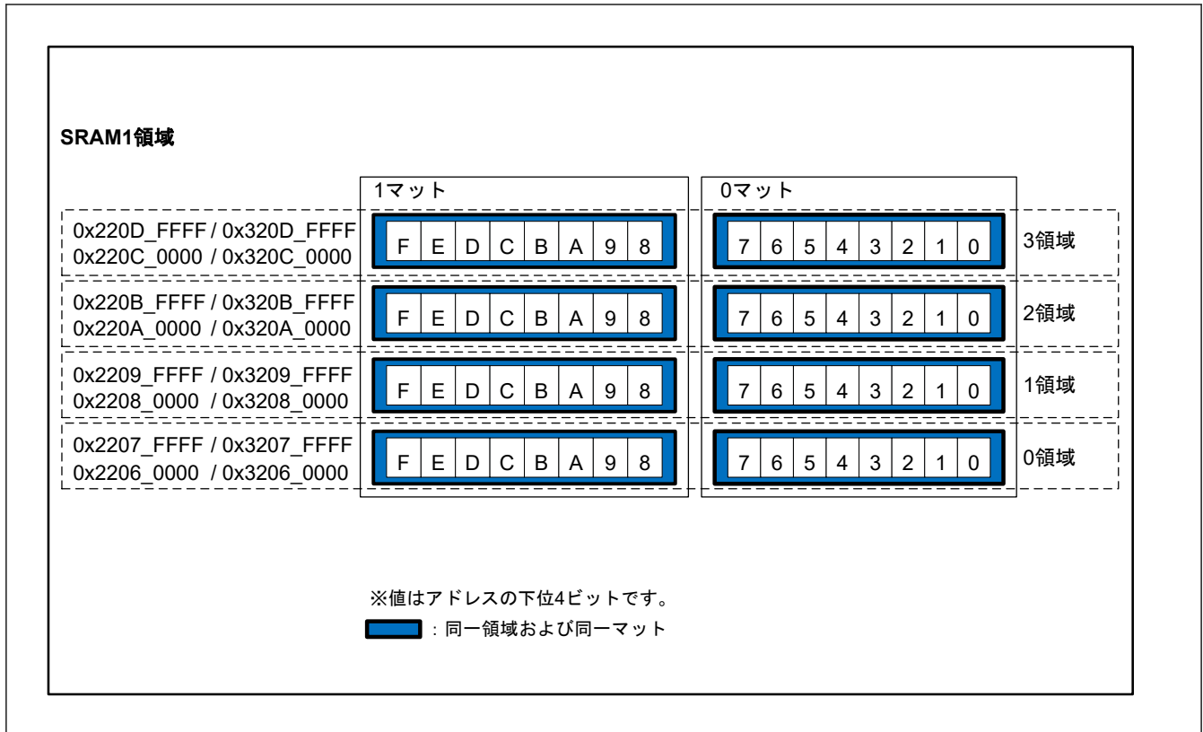
図 47.1 SRAM のマット設定
