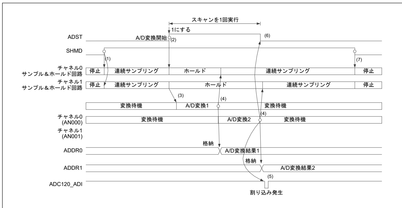
図 42.10 シングルスキャンモードの動作例 (チャンネル専用サンプル&ホールド回路使用、AN000 および AN001 選択、連続サンプリング有効)
