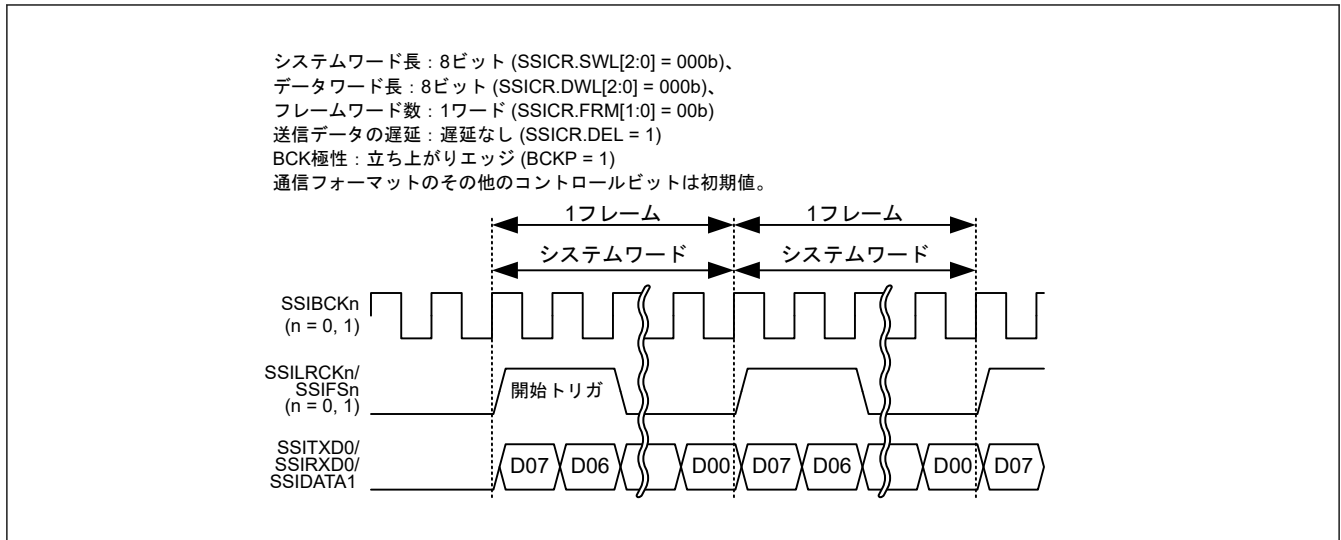
図 37.40 モノラルフォーマットにおけるロングフレーム (パディングなし)
