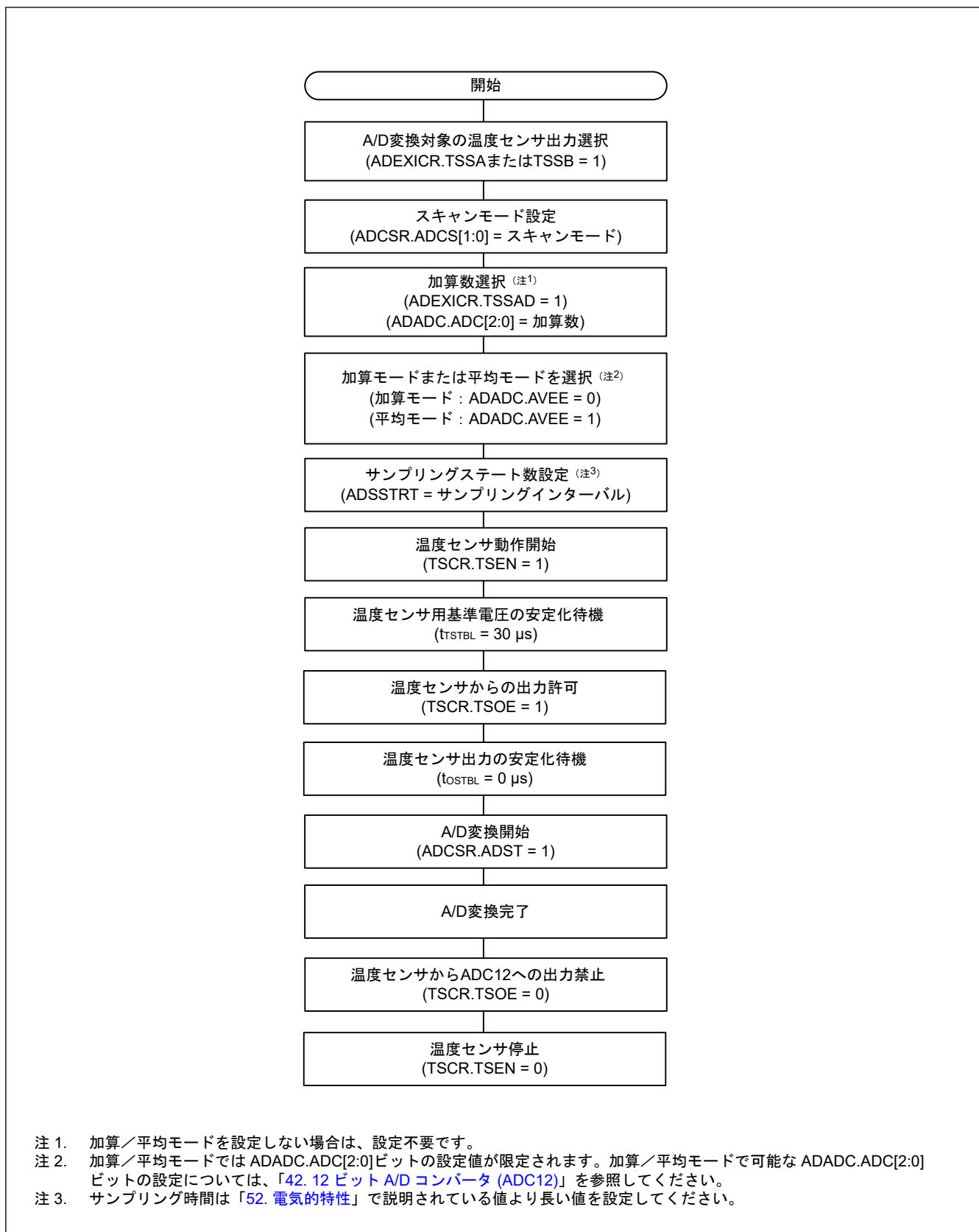
図 44.2 TSN の使用手順例
