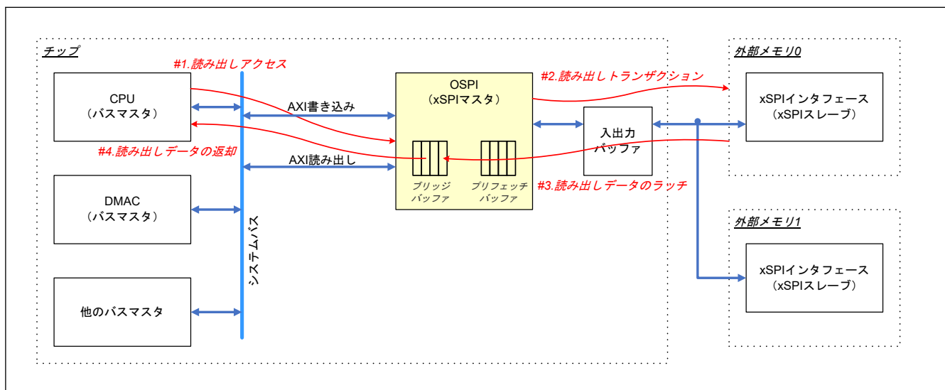
図 35.16 メモリ領域に対する読み出しアクセス
