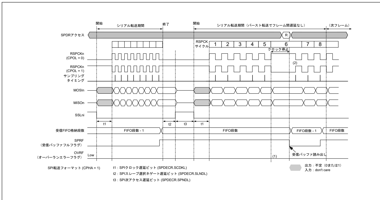
図 34.50 FIFO の段数分のデータが格納された受信バッファの状態でのシリアル転送が継続する場合のクロック停止波形 (バースト転送でフレーム間遅延なし、CPHA = 1)
