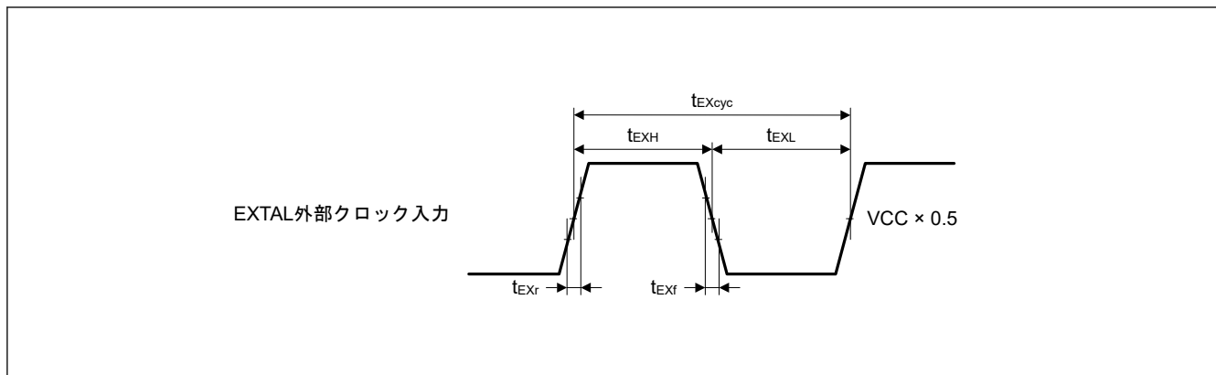
図 52.15 EXTAL 外部クロック入力タイミング
