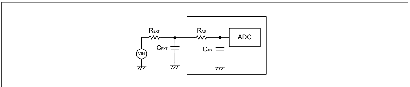
図 42.45 サンプル&amp;ホールド回路の簡略図
