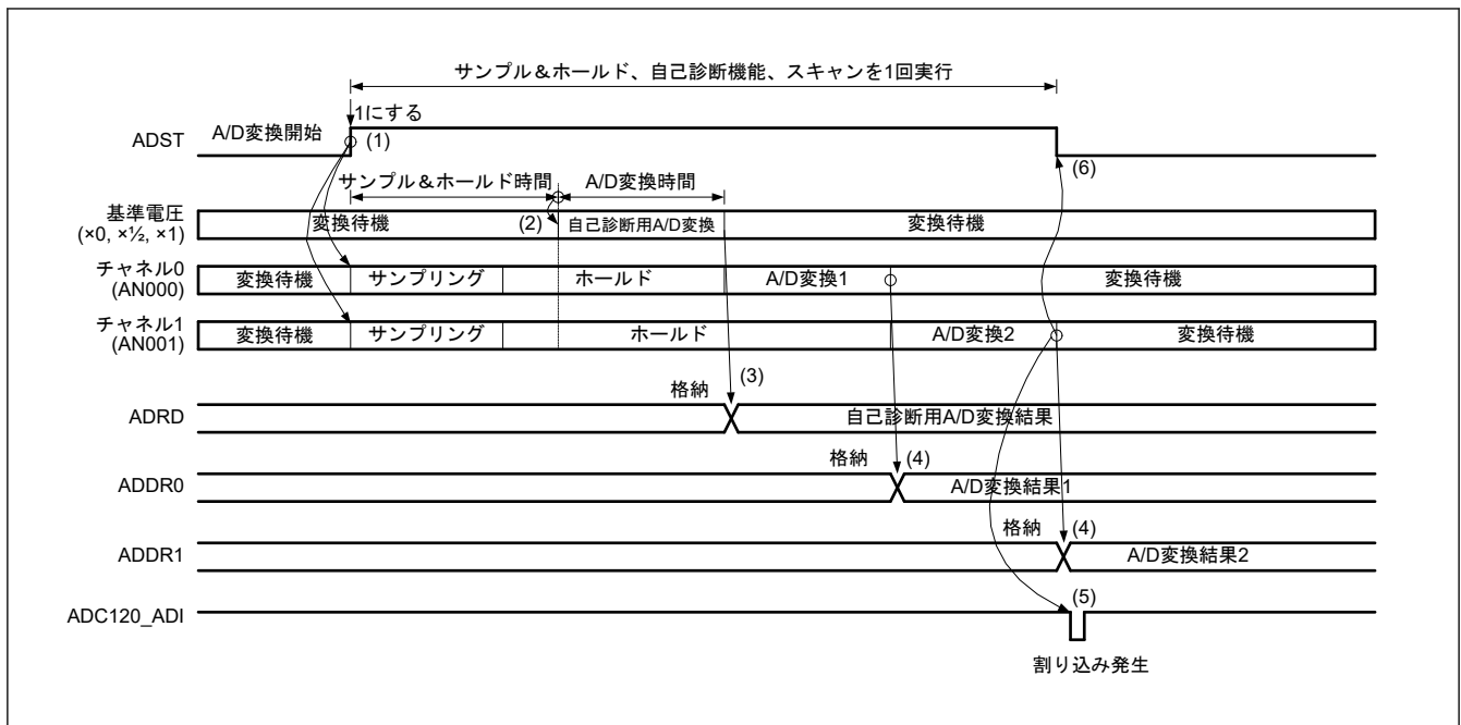
図 42.12 シングルスキャンモードの動作例（チャンネル専用サンプル&ホールド回路使用、自己診断で AN000, AN001 選択、連続サンプリング無効）
