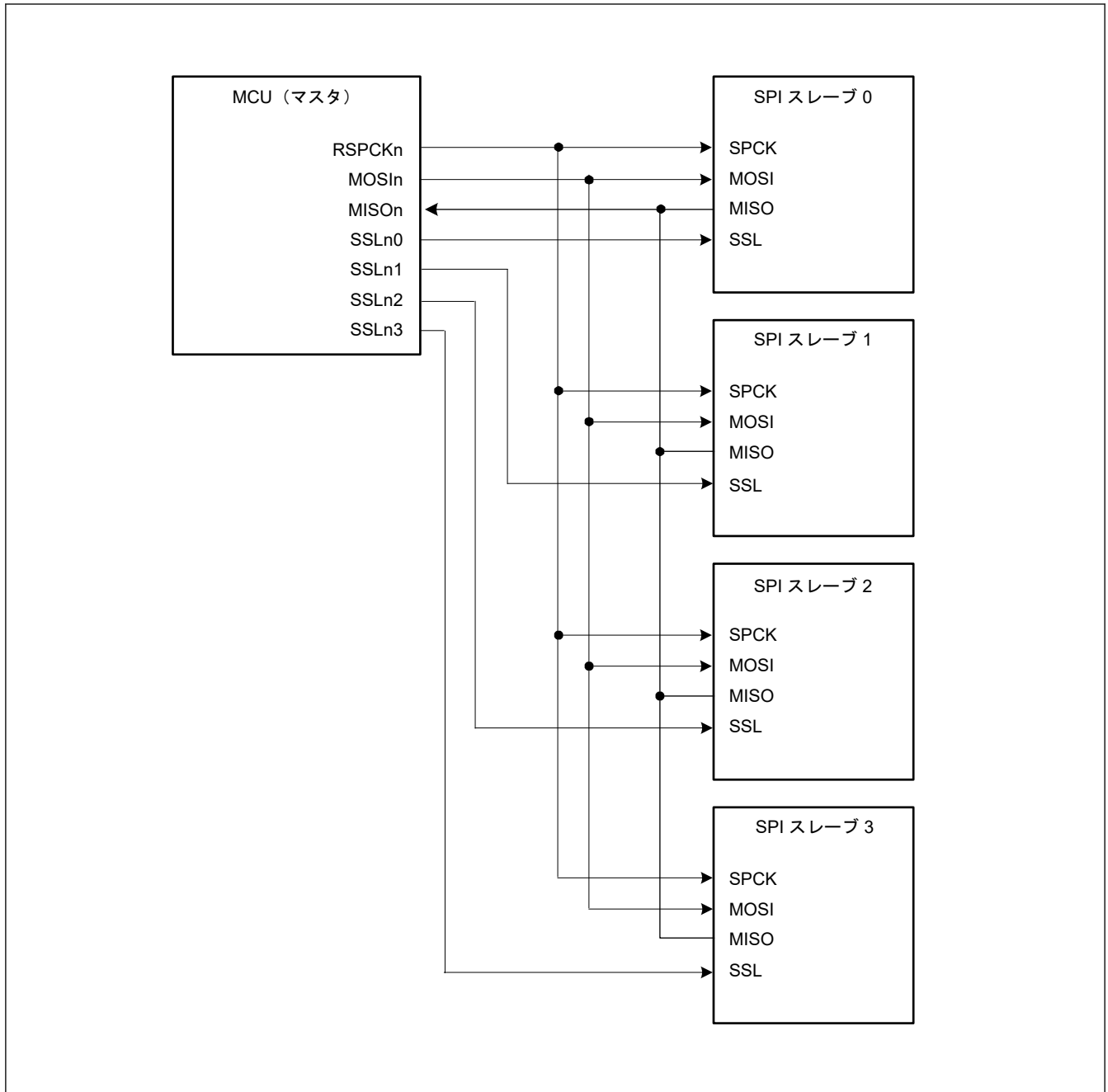
図 34.9 シングルマスタとマルチスレーブの構成例 (MCU はマスタ)
