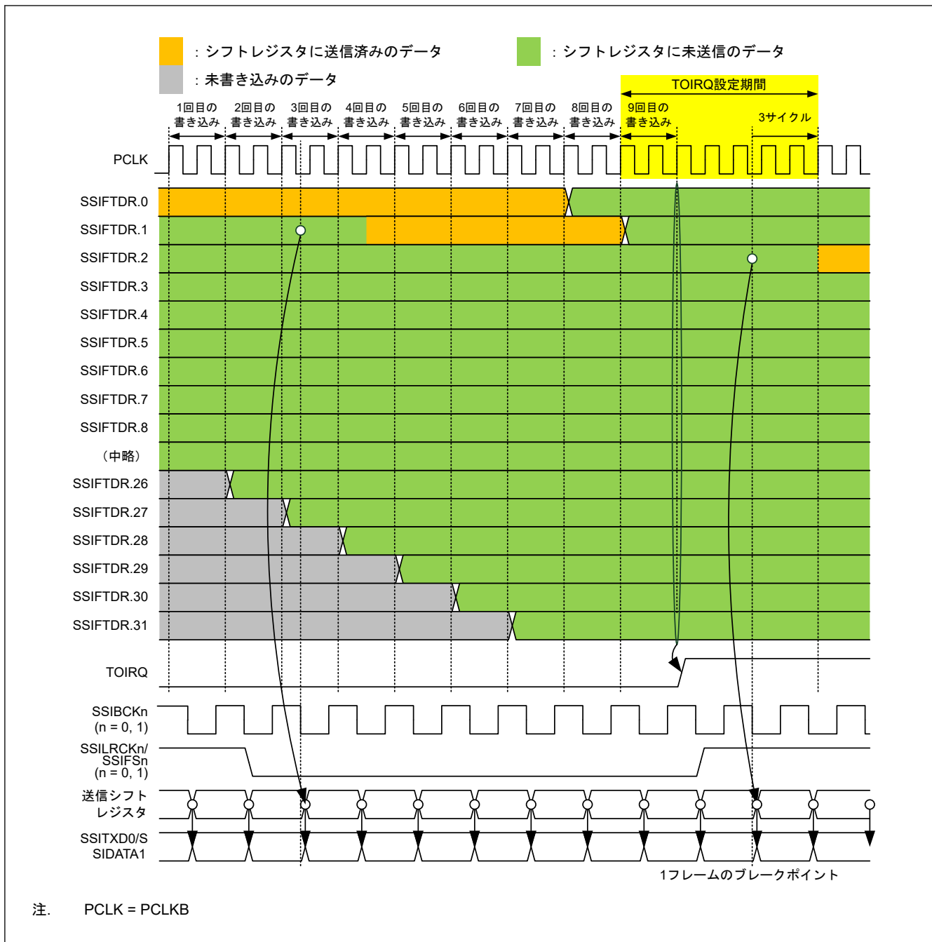
図 37.18 TOIRQ 設定タイミング
