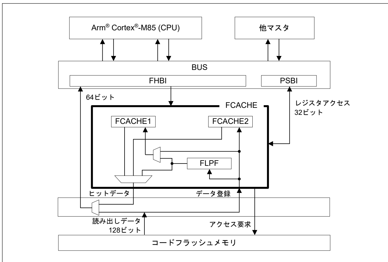
図 49.5 FCACHE のブロック図
