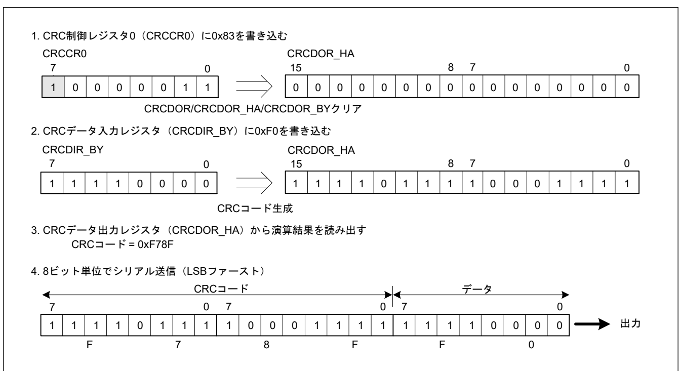
図 38.2 LSB ファーストのデータ送信
