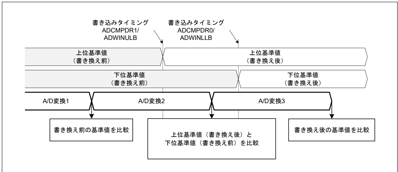
図 42.6 書き換え前後の上側基準値と下側基準値の比較
