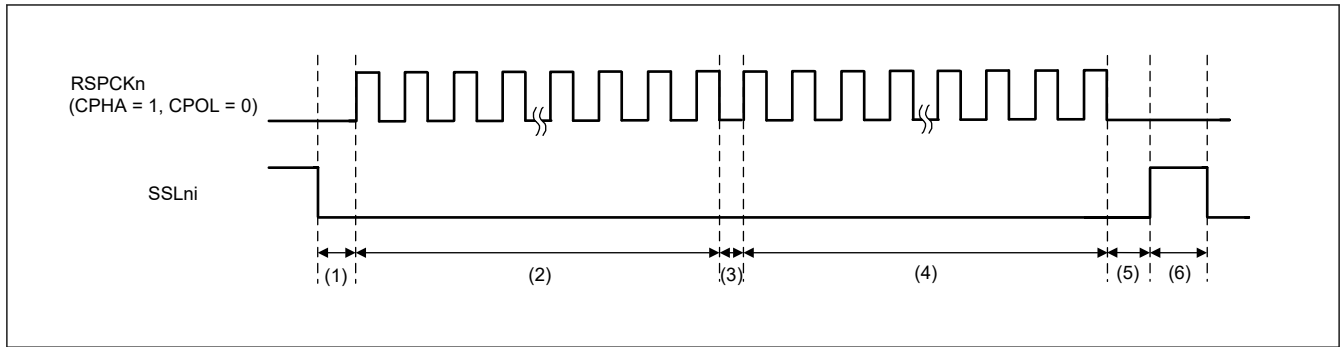
図 34.58 SSLKP ビットを利用したバースト転送の動作例 (BFDS = 1、SPFRF = 0)
