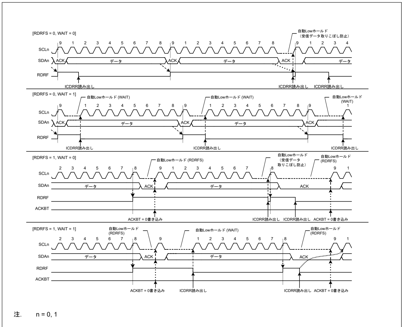
図 31.40 受信モード時の自動 Low ホールド動作 (RDRFS および WAIT ビットを使用)
