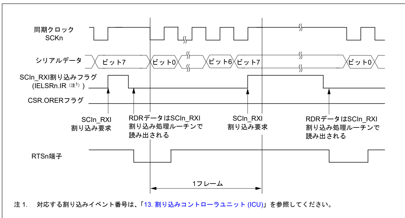
図 30.68 クロック同期式モードにおけるシリアル受信の動作例 (2) (RTS 機能を使用する場合)
