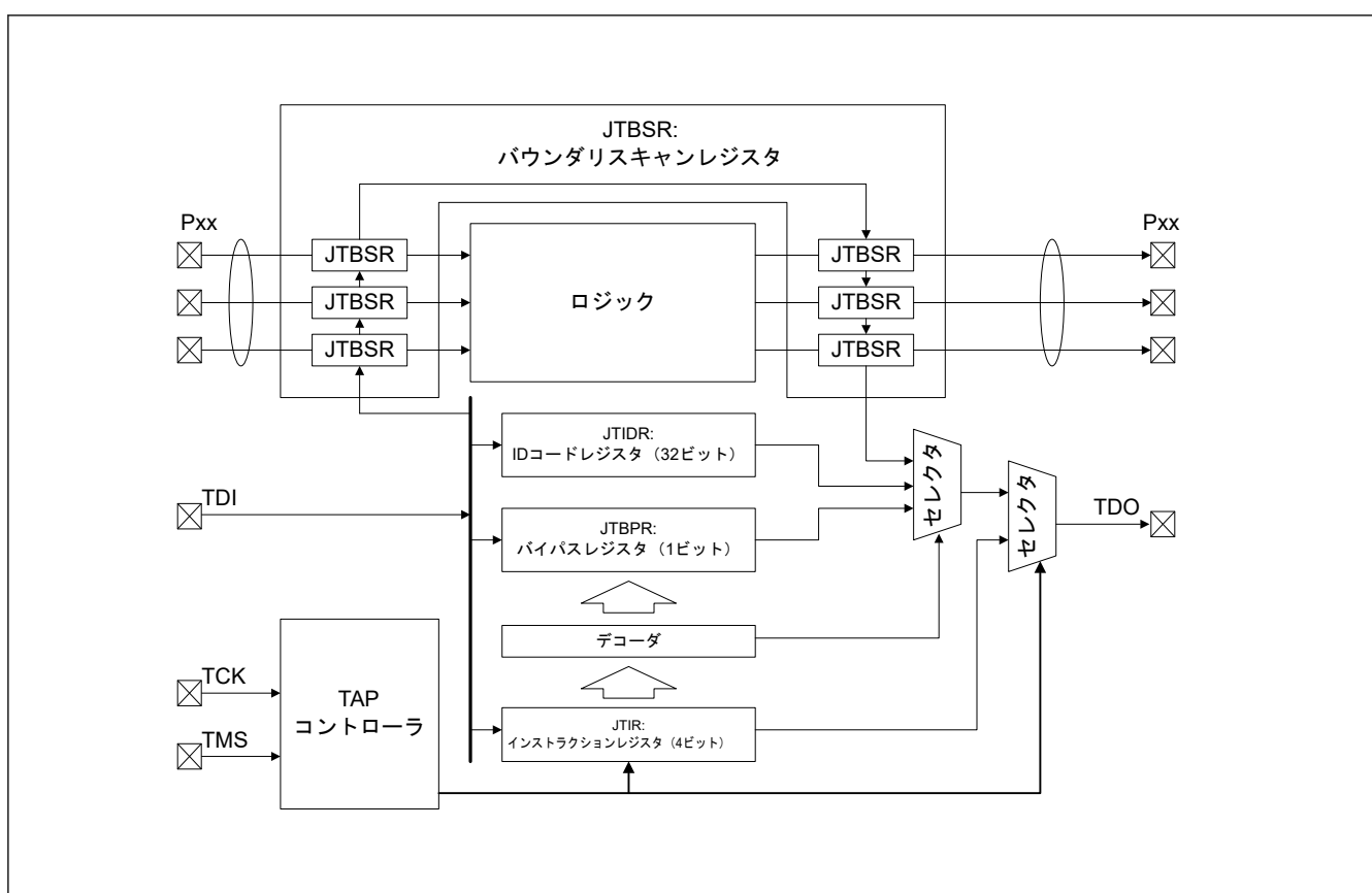
図 39.1 バウンダリスキャン機能のブロック図
