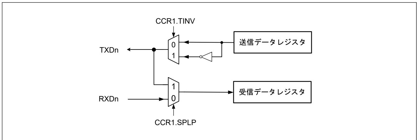
図 30.115 ループバックモードでのシフトレジスタの入出力構成イメージ
