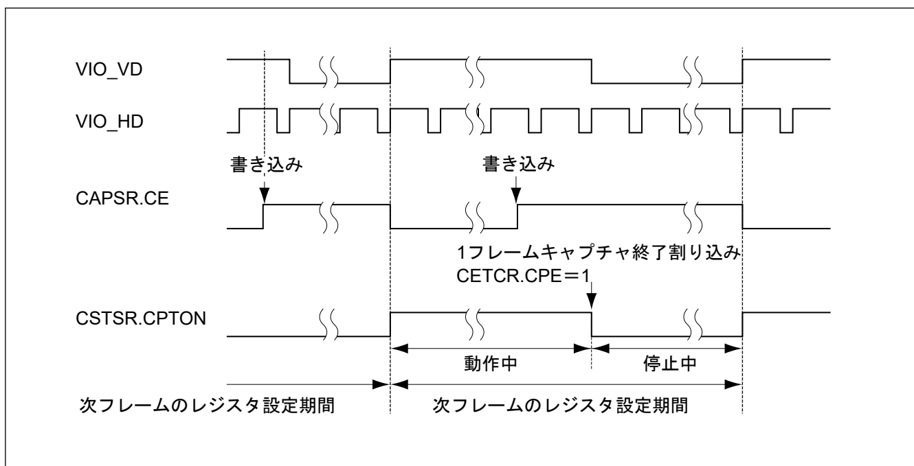
図 50.7 1 フレームキャプチャの CE ビット書き込みタイミングとレジスタ設定
