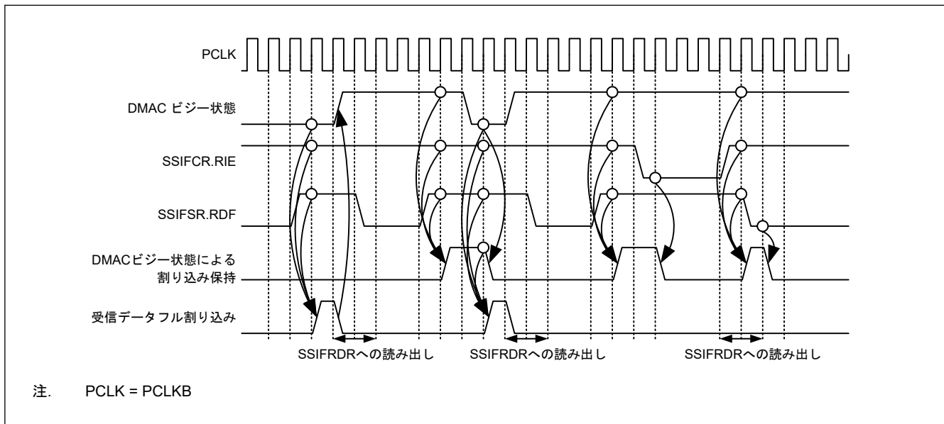
図 37.22 受信データフル割り込みのタイミング
