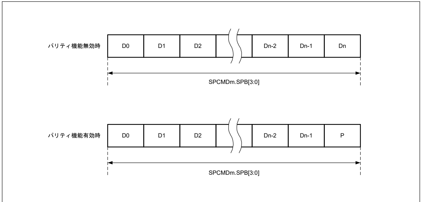
図 34.14 パリティ機能無効時と有効時のデータフォーマット
