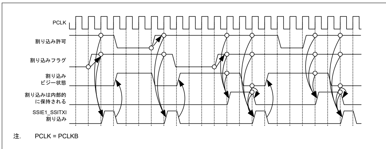
図 37.60 SSIE1_SSITXI 割り込みタイミング図
