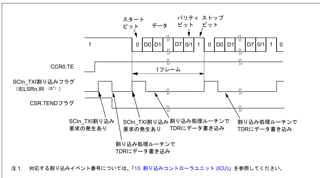
図 30.12 調歩同期式モードにおけるシリアル送信の動作例 (1) (8 ビットデータ/パリティあり/1 ストップビット/CTS 機能不使用/送信開始時)
