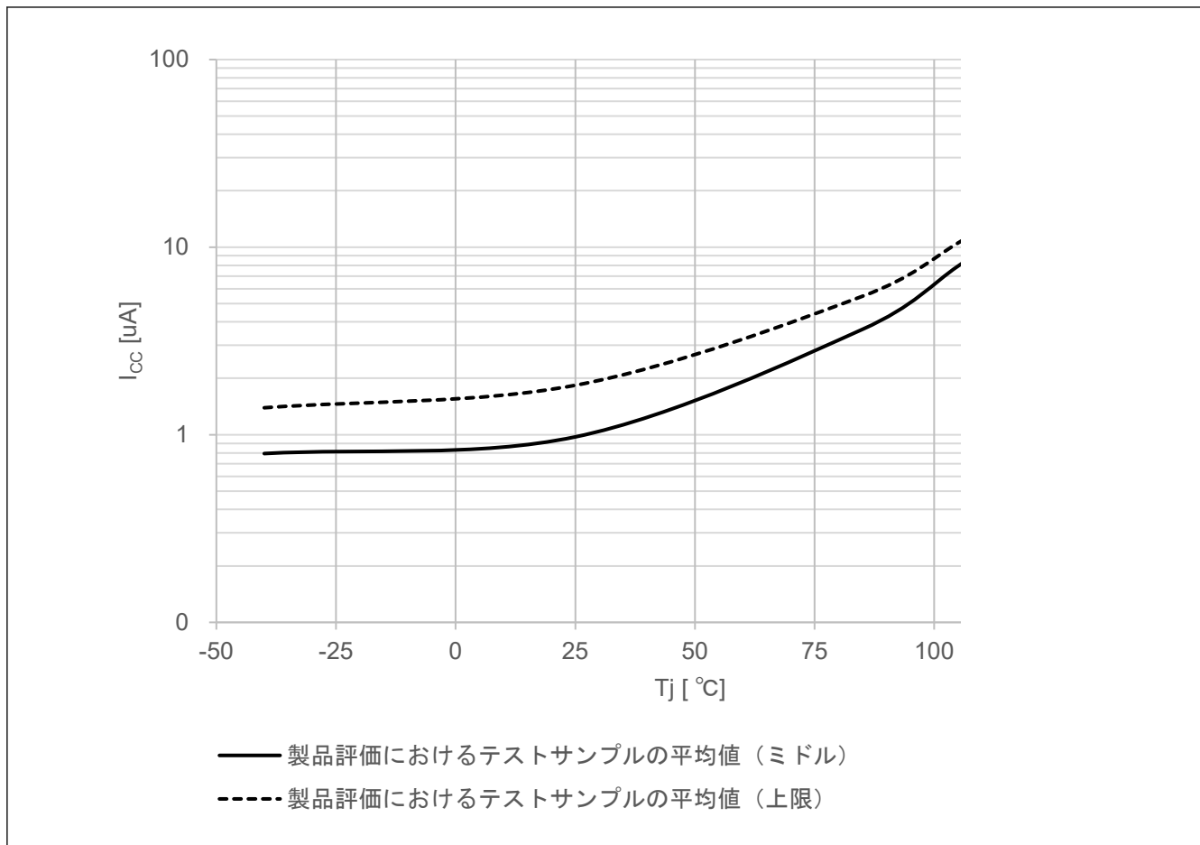
図 52.7 ディープソフトウェアスタンバイモード3における温度依存性 (参考データ)
