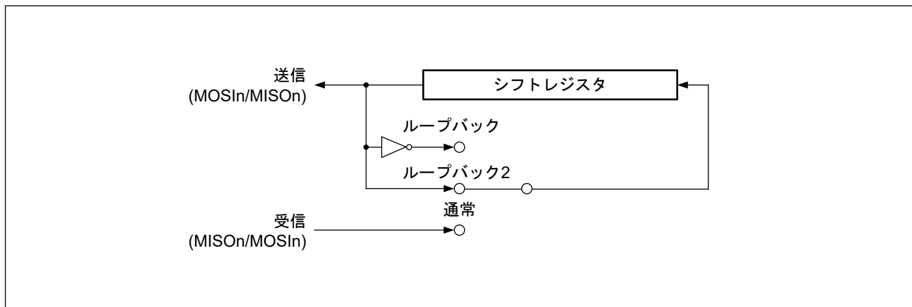
図 34.78 ループバックモード時のシフトレジスタ入出力経路の構成 (マスターモード)
