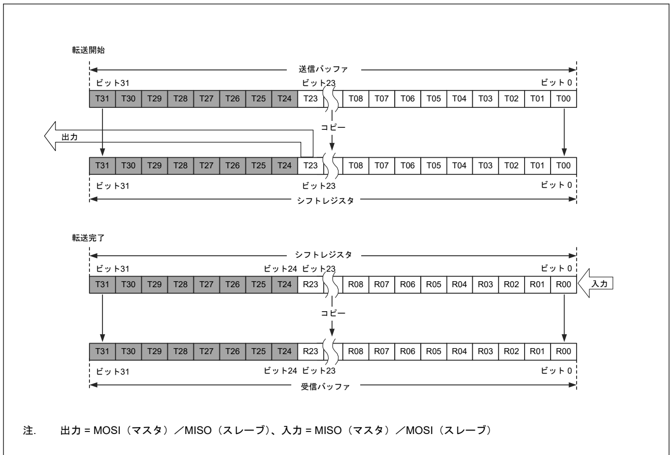
図 34.16 MSB ファースト転送 (24 ビットデータ/パリティ機能無効)
