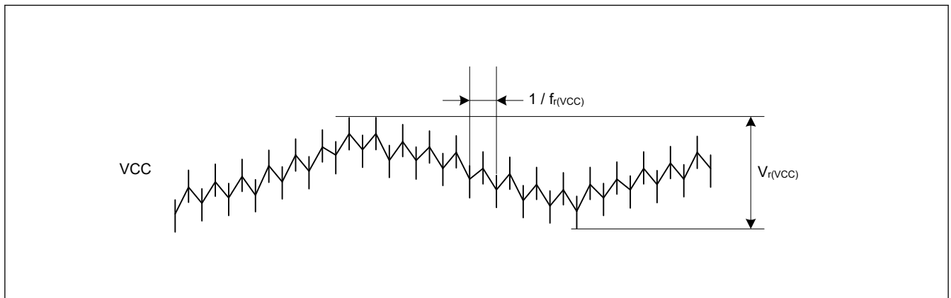
図 52.13 リップル波形
