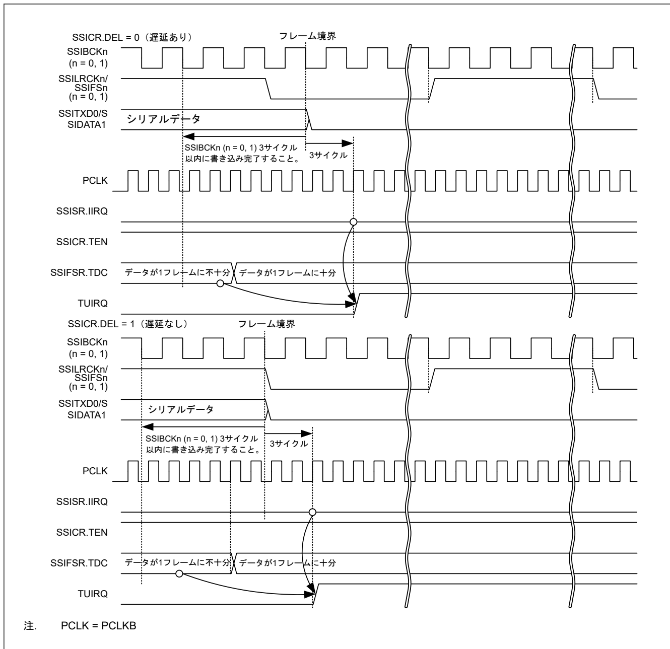
図 37.20 TUIRQ 設定タイミング (通信継続時)
