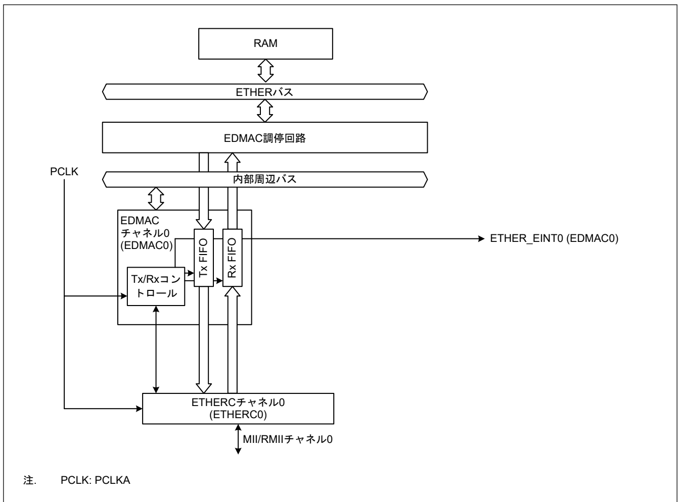
図 28.1 EDMAC の構成
