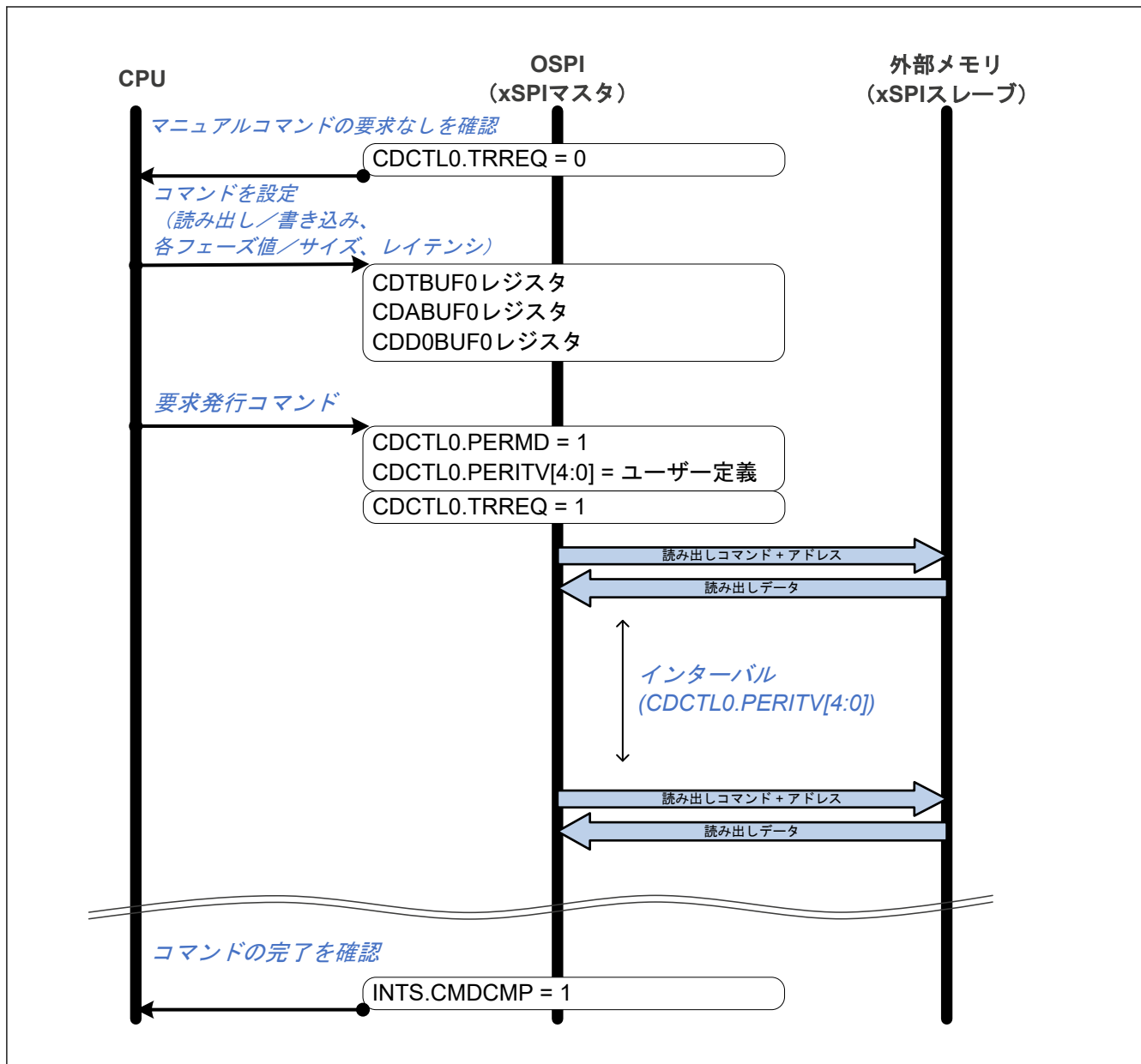
図 35.26 マニュアルコマンド手順のフロー (周期モード)
