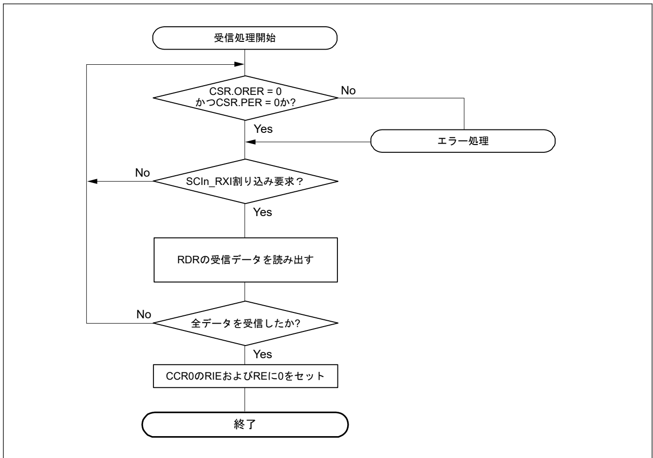
図 30.84 スマートカードインタフェース受信のフローチャート例
