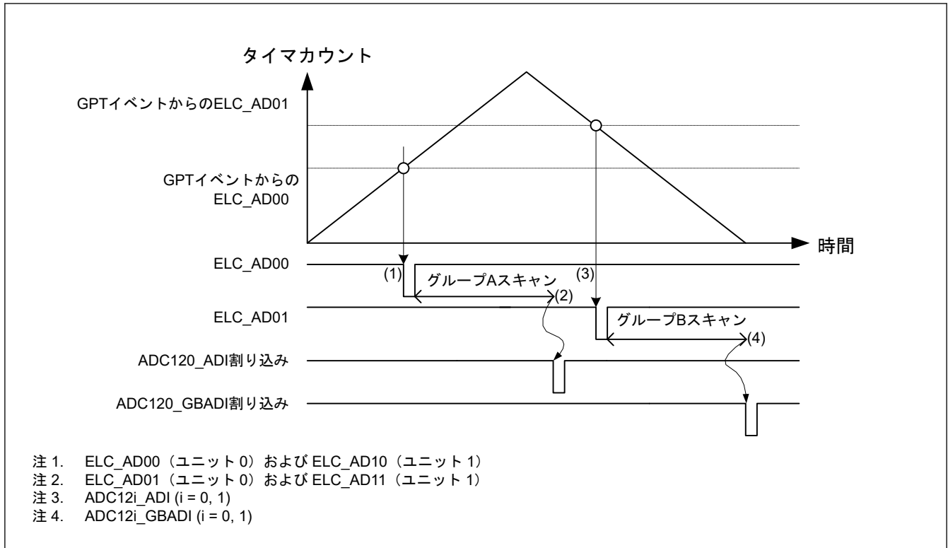
図 42.24 グループスキャンモードの基本動作例 (ELC からの同期トリガ使用)
