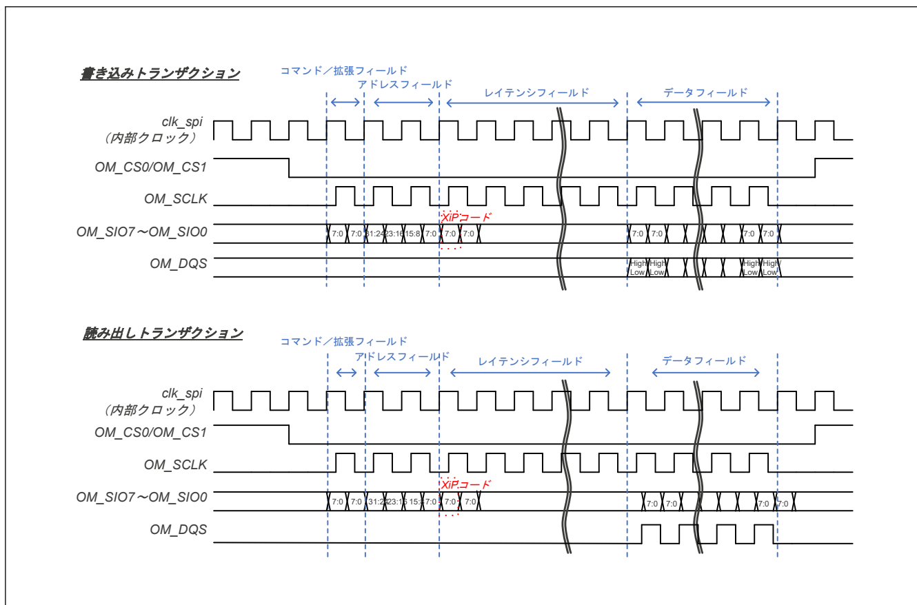
図 35.6 8D-8D-8D プロファイル 1.0 のタイミングチャート
