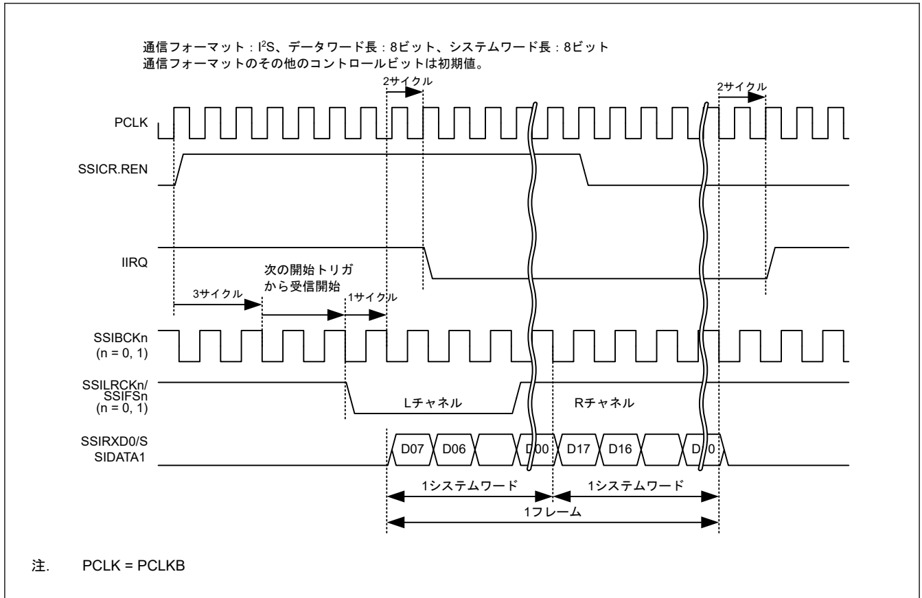
図 37.15 IIRQ 設定タイミング (受信)
