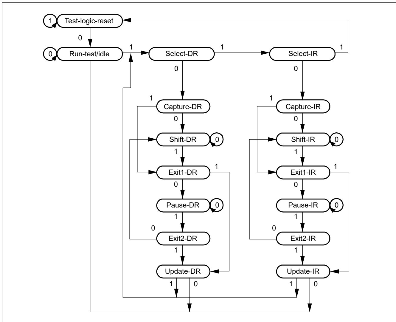
図 39.2 TAP コントローラの状態遷移図
