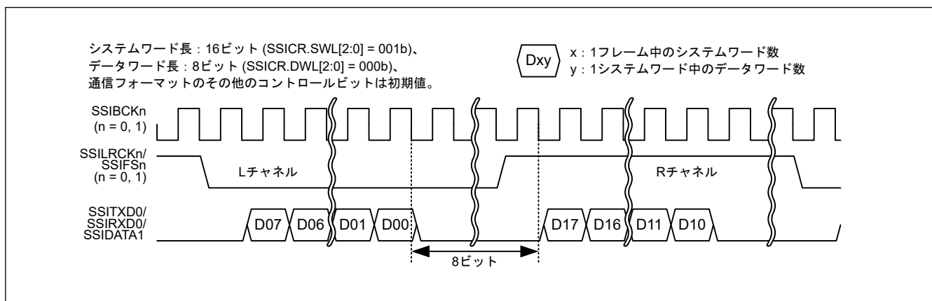
図 37.36 パディングビット転送の例 (I 2 S フォーマット、システムワード長 > データワード長)
