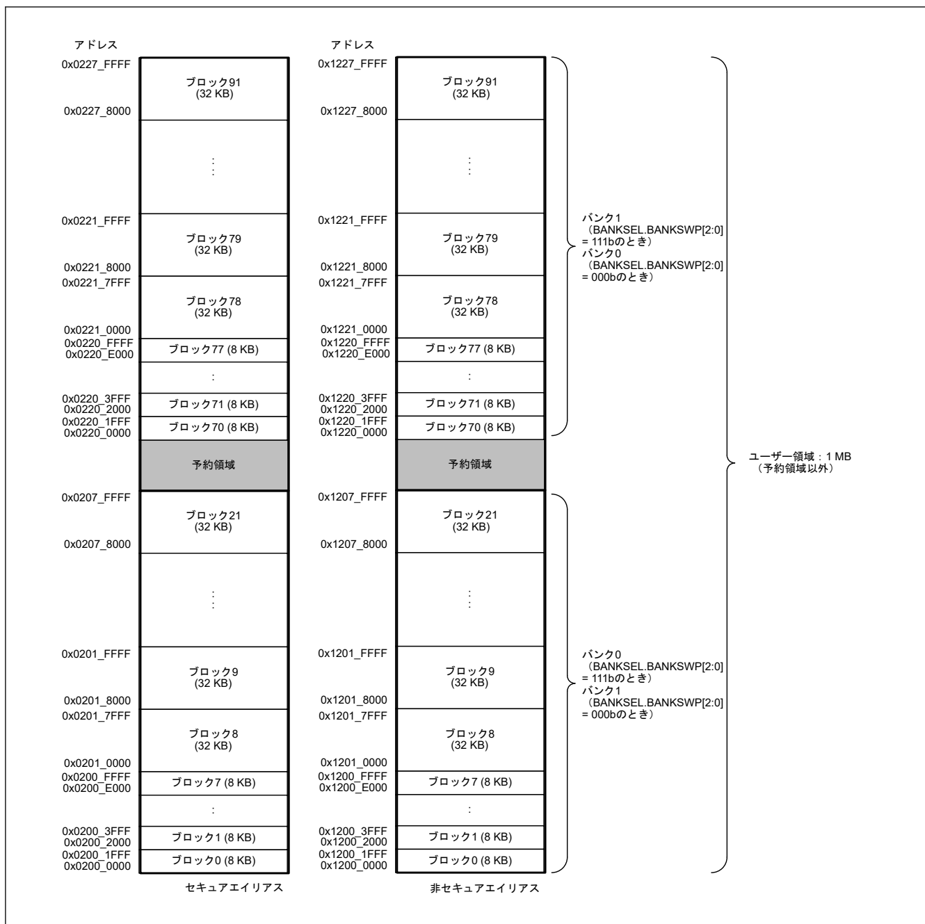
図 49.3 デュアルモードでのコードフラッシュメモリのマップ
