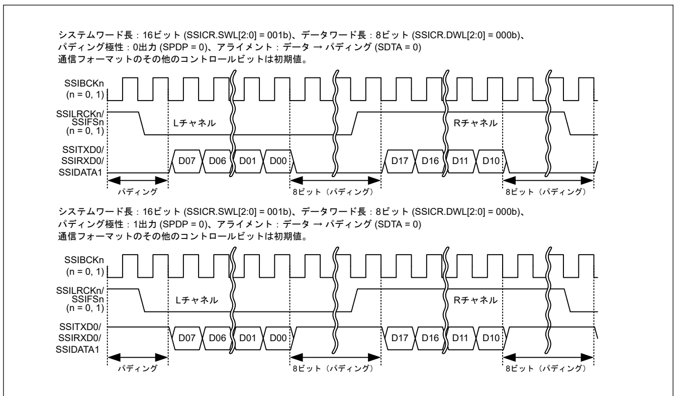
図 37.11 パディングビットの極性
