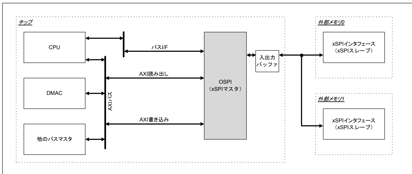
図 35.1 ブロック図
