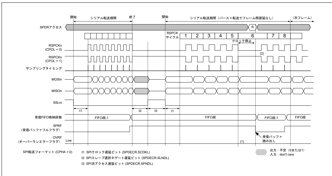
図 34.51 マスタモードにおいて FIFO の段数分のデータが格納された状態でシリアル転送が継続する場合のクロック停止波形 (バースト転送でフレーム間遅延なし、CPHA = 0)
