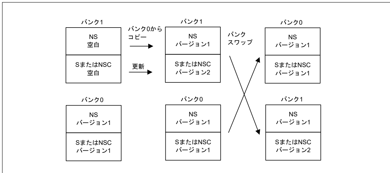
図 40.11 セキュア領域または NSC 領域のフィールドアップデートフロー
