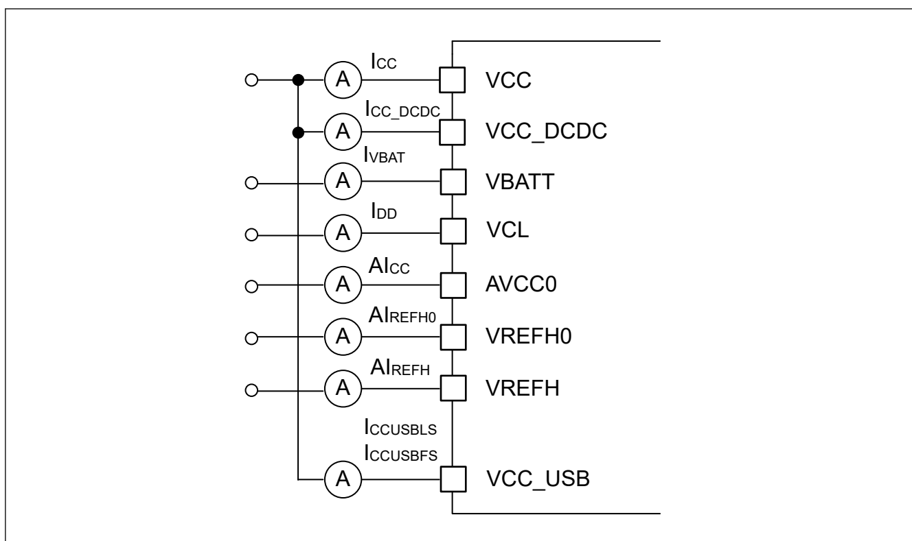
図 52.2 消費電流測定図
