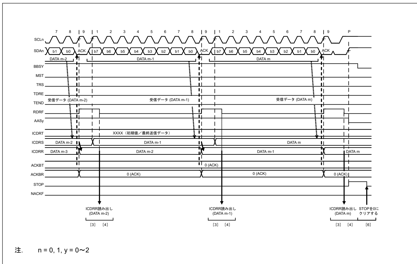
図 31.20 スレープ受信の動作タイミング (2) (RDRFS = 0の場合)
