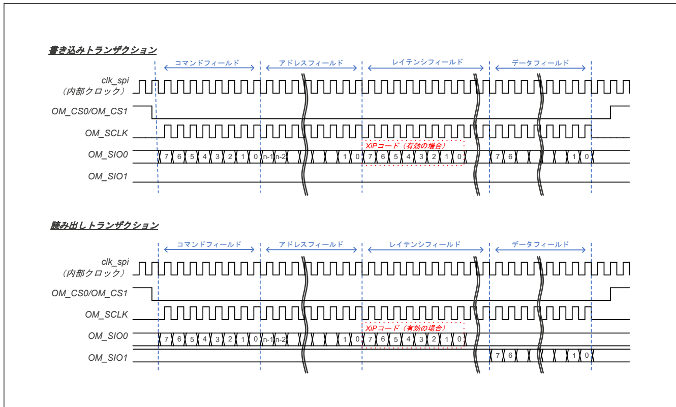
図 35.3 1S-1S-1S のタイミングチャート
