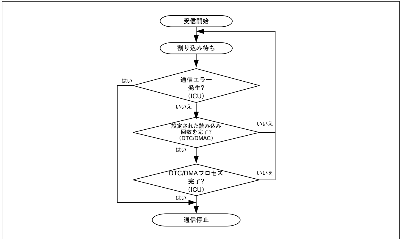
図 37.55 受信手順
