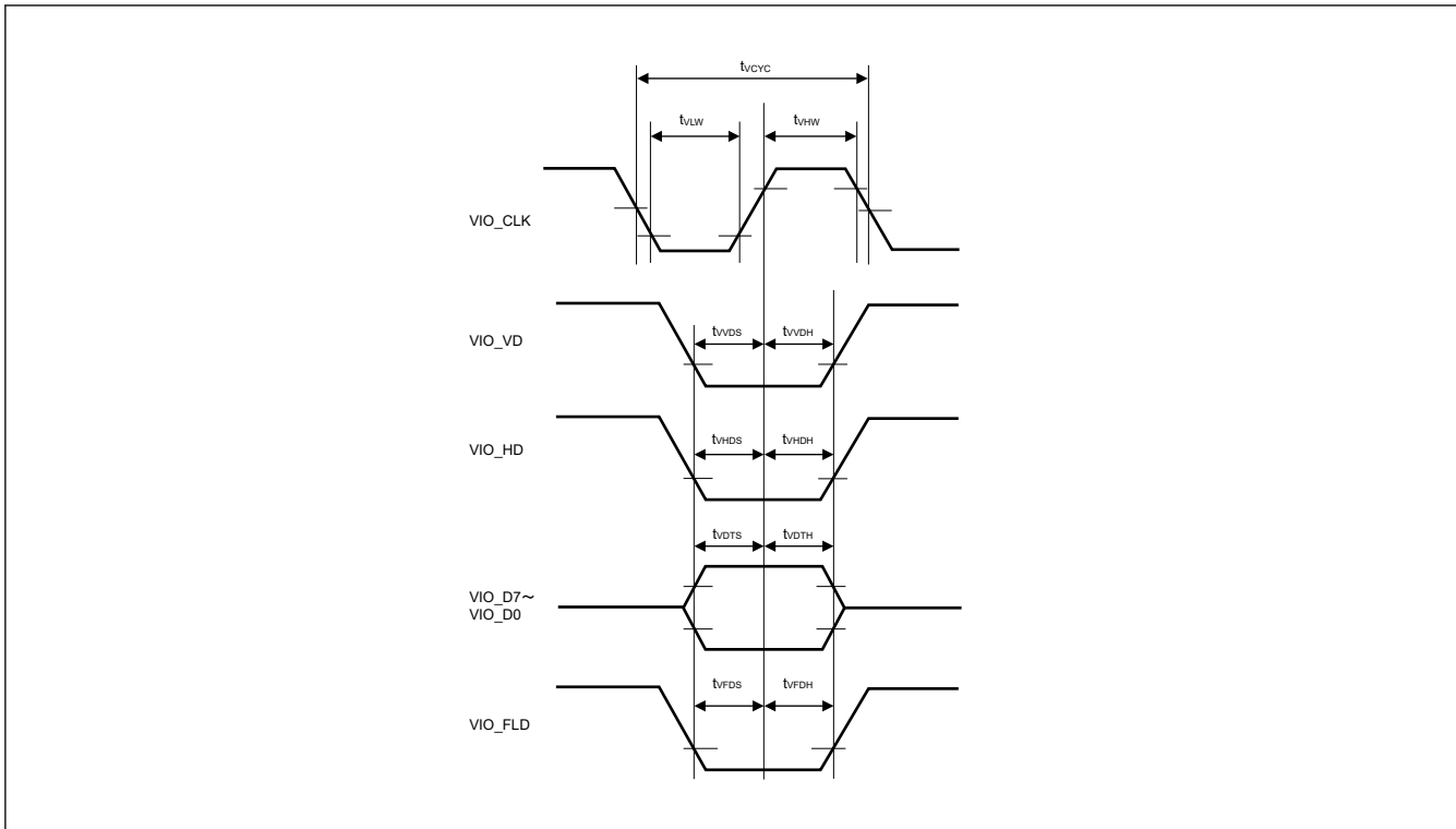
図 52.71 VIO_CLK の立ち上がりエッジによるデータキャプチャのキャプチャエンジンユニットモジュール信号タイミング
