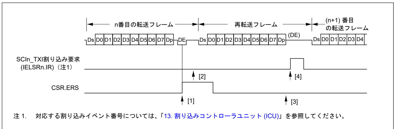
図 30.80 スマートカードインタフェース送信モードでのデータ再送信動作
