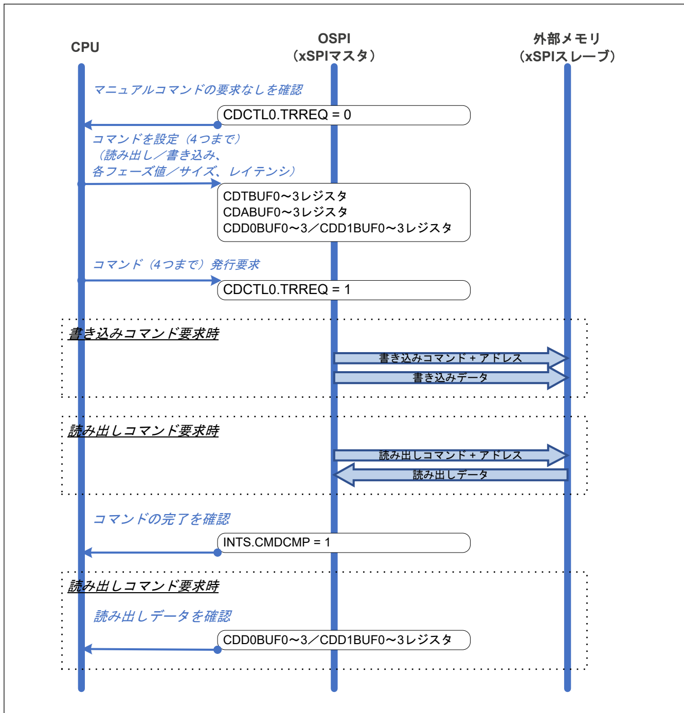
図 35.25 マニュアルコマンド手順のフロー (直接モード)
