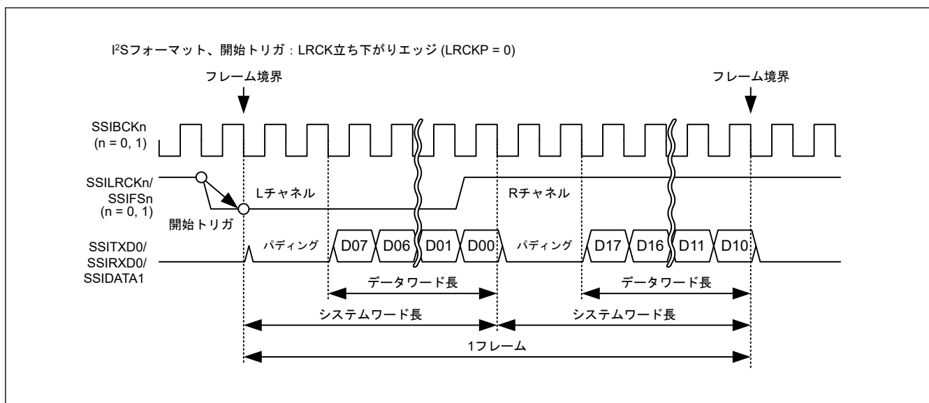
図 37.1 通信フォーマットの定義
