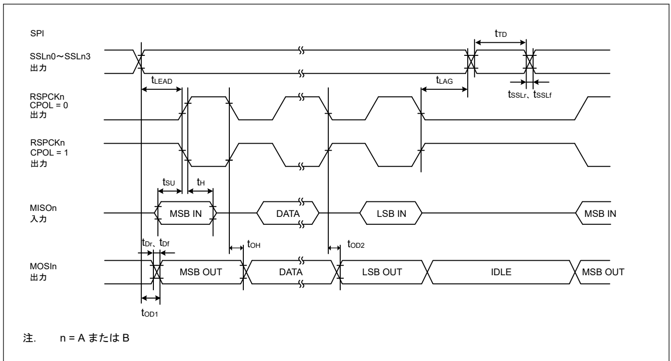
図 52.43 CPHA = 0 の場合におけるモトローラ SPI マスタの SPI タイミング
