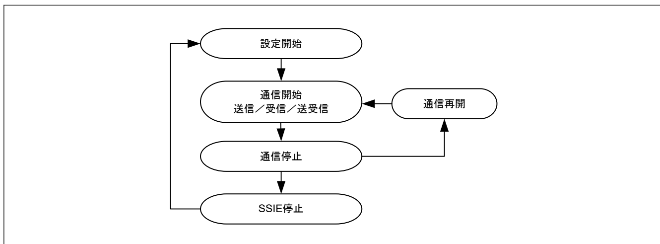
図 37.52 SSIE の通信動作
