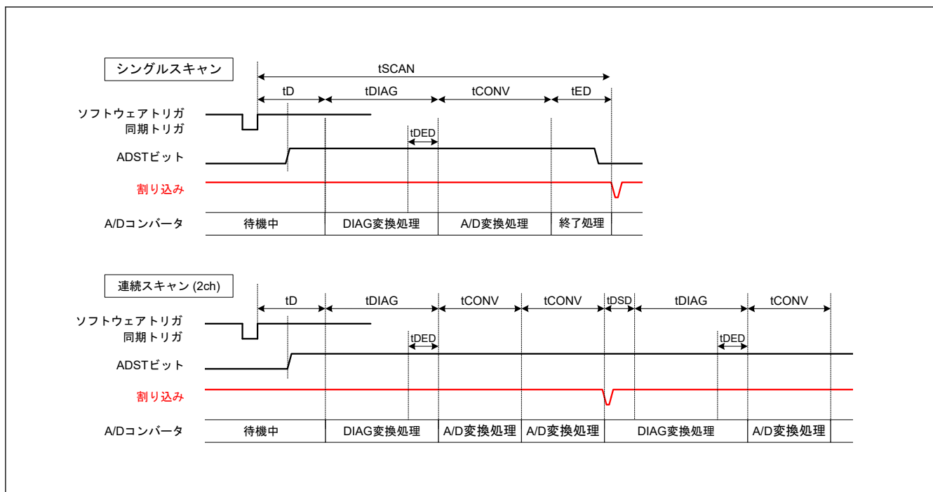
図 42.35 スキャン変換のタイミング (ソフトウェア起動または同期トリガ入力 (GPT, ELC) 起動の場合)
