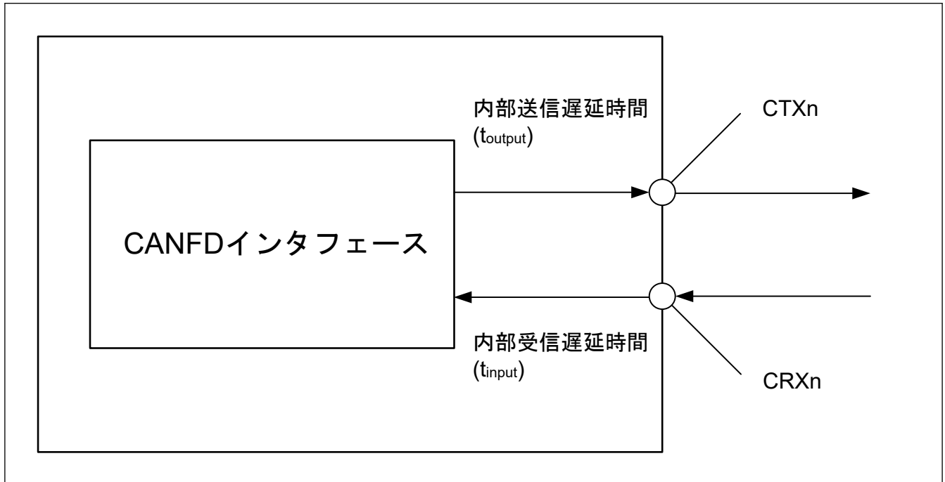
図 52.73 CANFD インタフェース条件
