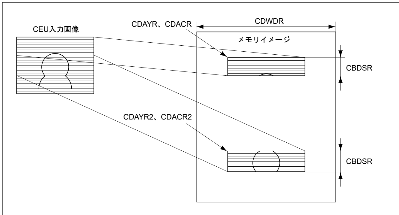
図 50.41 バンドル書き込みメモリ格納イメージ
