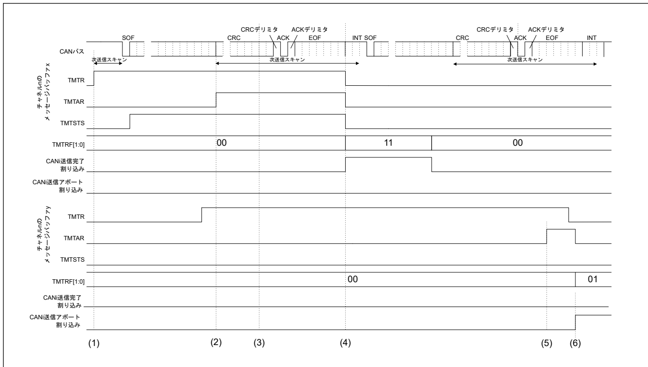
図 32.44 送信アボートの要求およびフラグビットのタイミング
