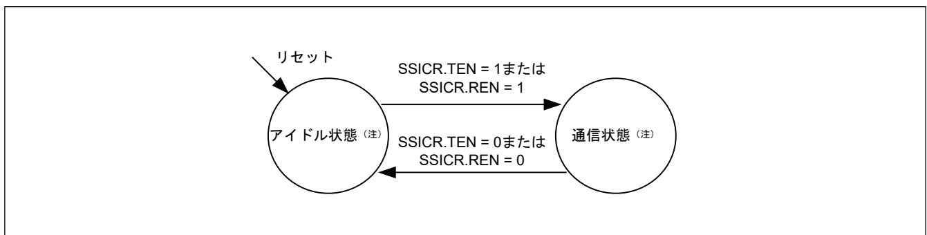
図 37.43 SSIE の状態遷移
