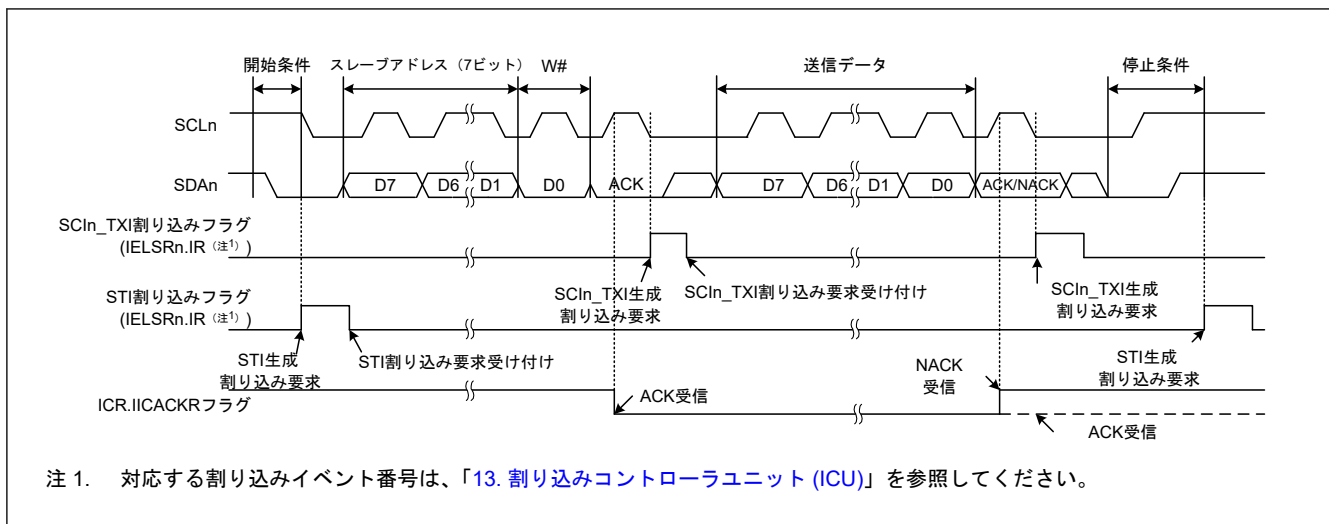
図 30.91 簡易 IIC モードにおけるマスタ送信の動作例 1 (7 ビットスレーブアドレス、送信割り込み、受信割り込み使用時) (ICR.IICINTM = 1)
