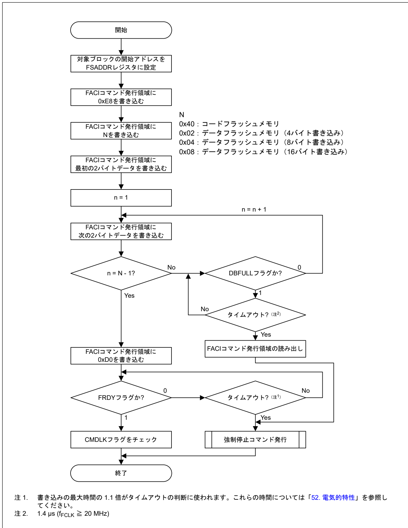
図 49.14 プログラムコマンドの使用フロー
