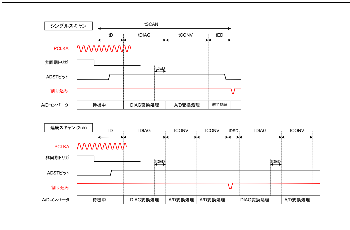
図 42.36 スキャン変換のタイミング (非同期トリガ入力 (ADTRGn (n = 0, 1)) 起動の場合)
