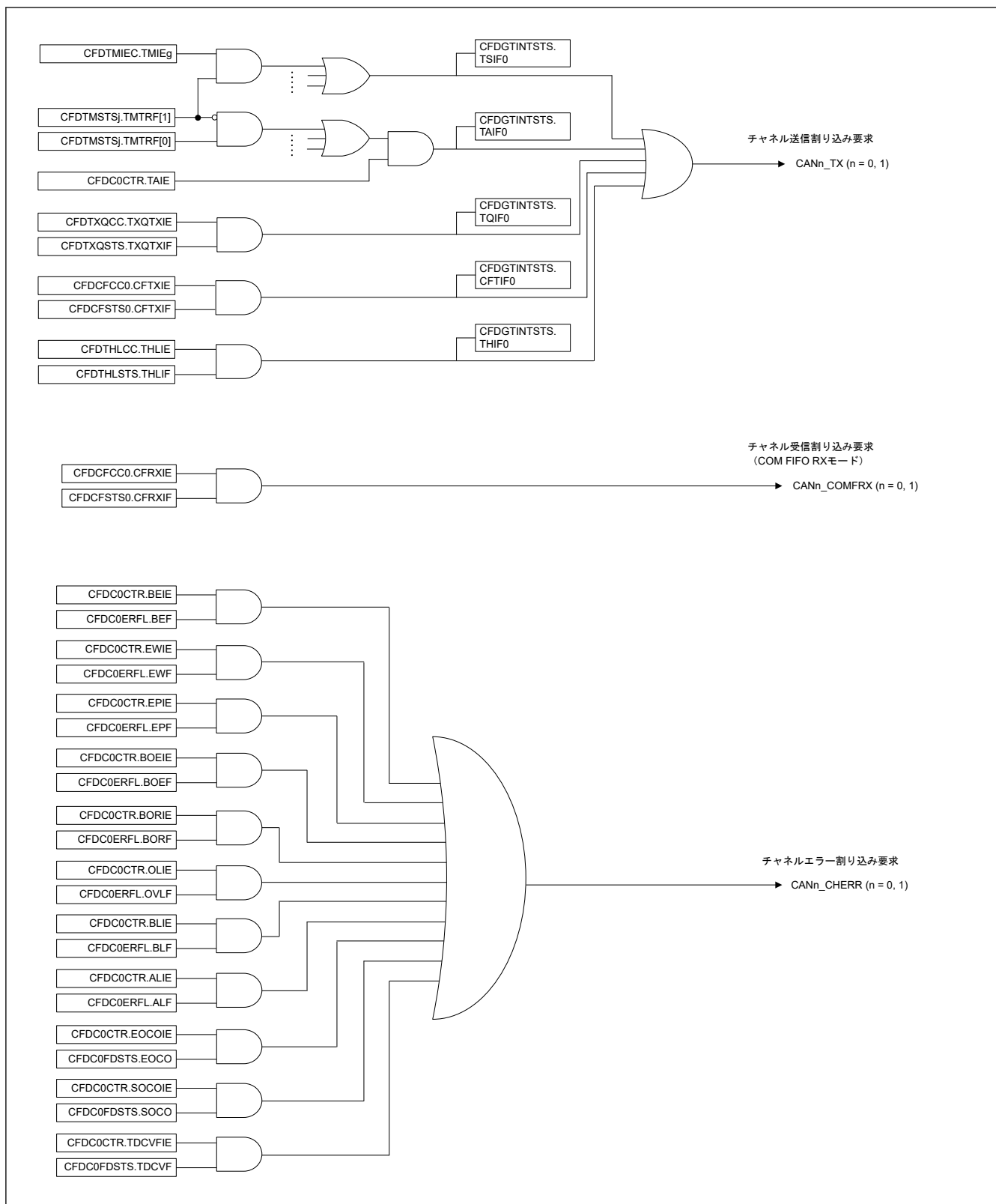
図 32.31 チャンネル割り込みのブロック図
