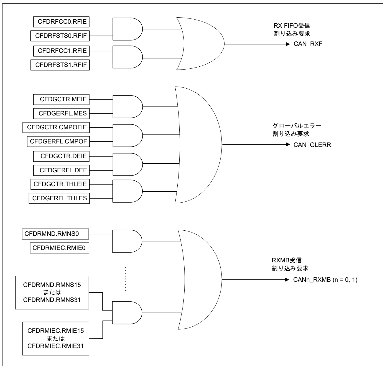
図 32.30 グローバル割り込みのブロック図
