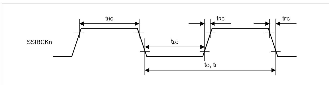
図 52.56 SSIE クロック入出力タイミング
