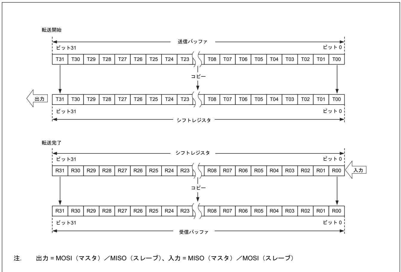
図 34.15 MSB ファースト転送 (32 ビットデータ/パリティ機能無効)
