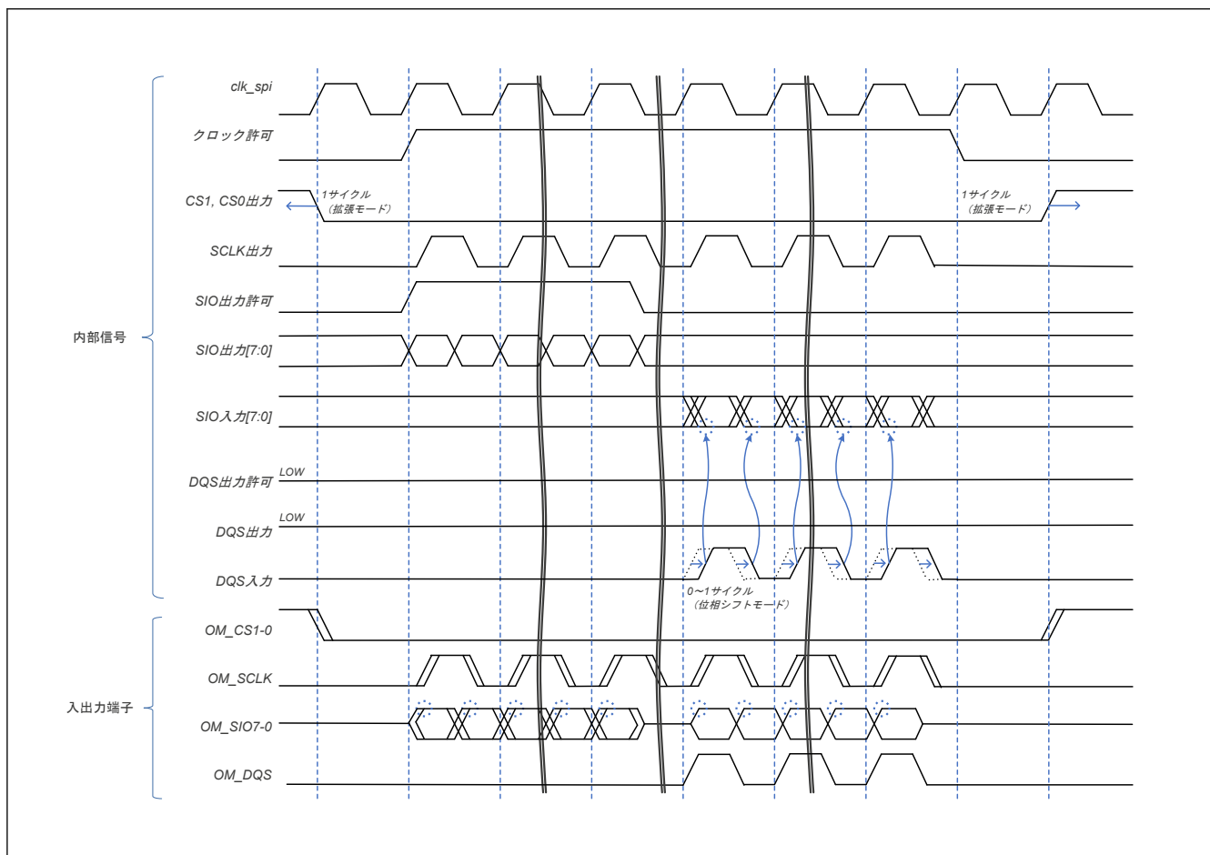
図 35.10 OM_DQS あり DDR のタイミング制御
