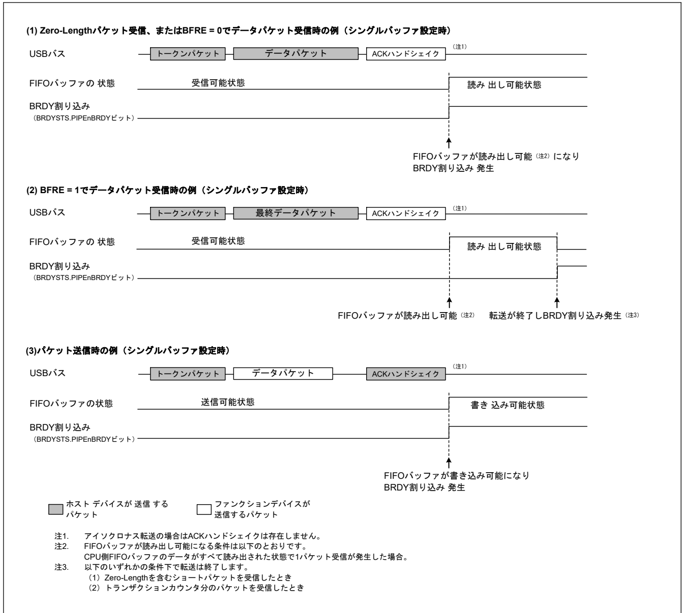
図 29.11 BRDY 割り込み発生タイミング
