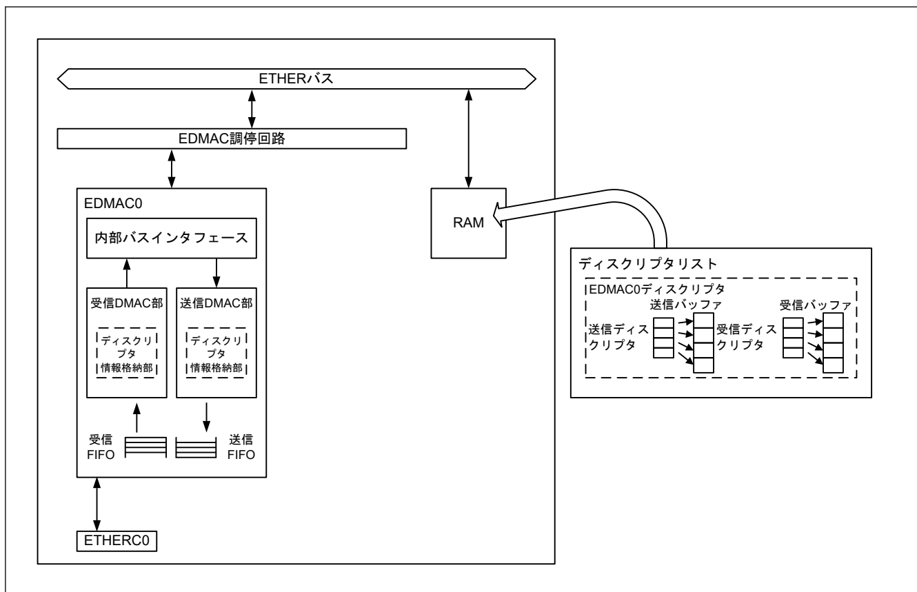
図 28.2 メモリ内のディスクリプタおよび送受信バッファの構成
