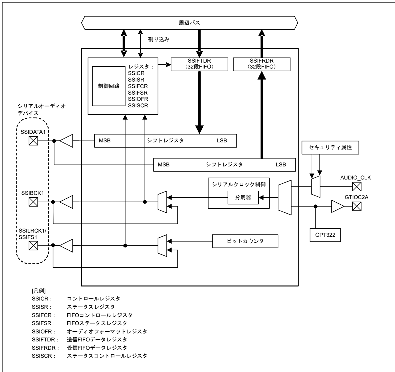
図 37.3 SSIE ブロック図 (SSIE1)
