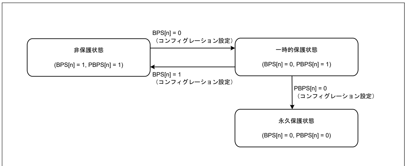
図 49.37 BPS[n]ビットおよび PBPS[n]ビットによるフラッシュシーケンサの状態遷移
