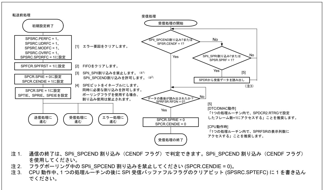
図 34.71 マスタモード時のソフトウェア処理フローチャート (受信のみ)
