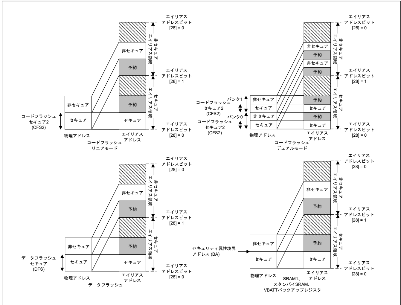
図 40.6 メモリマッピング
