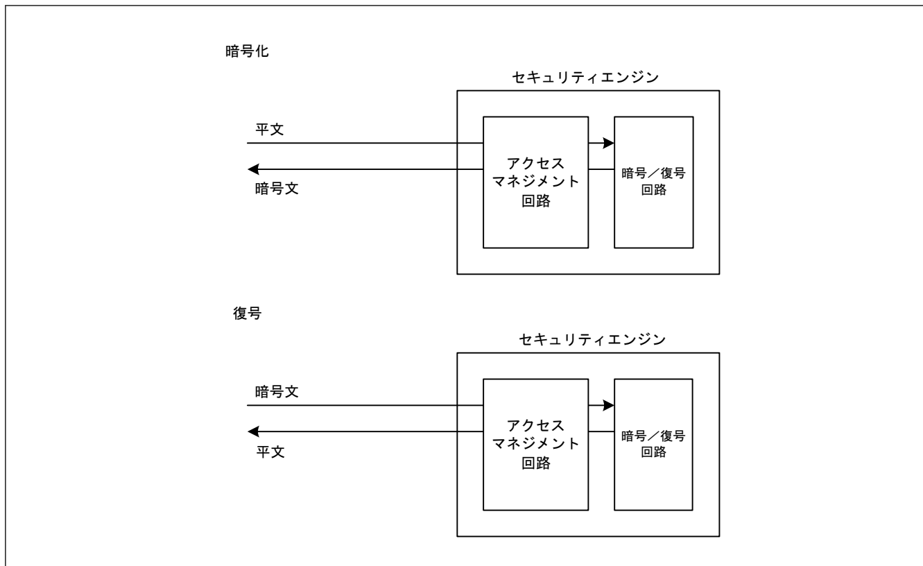
図 41.2 対称暗号の概念図
