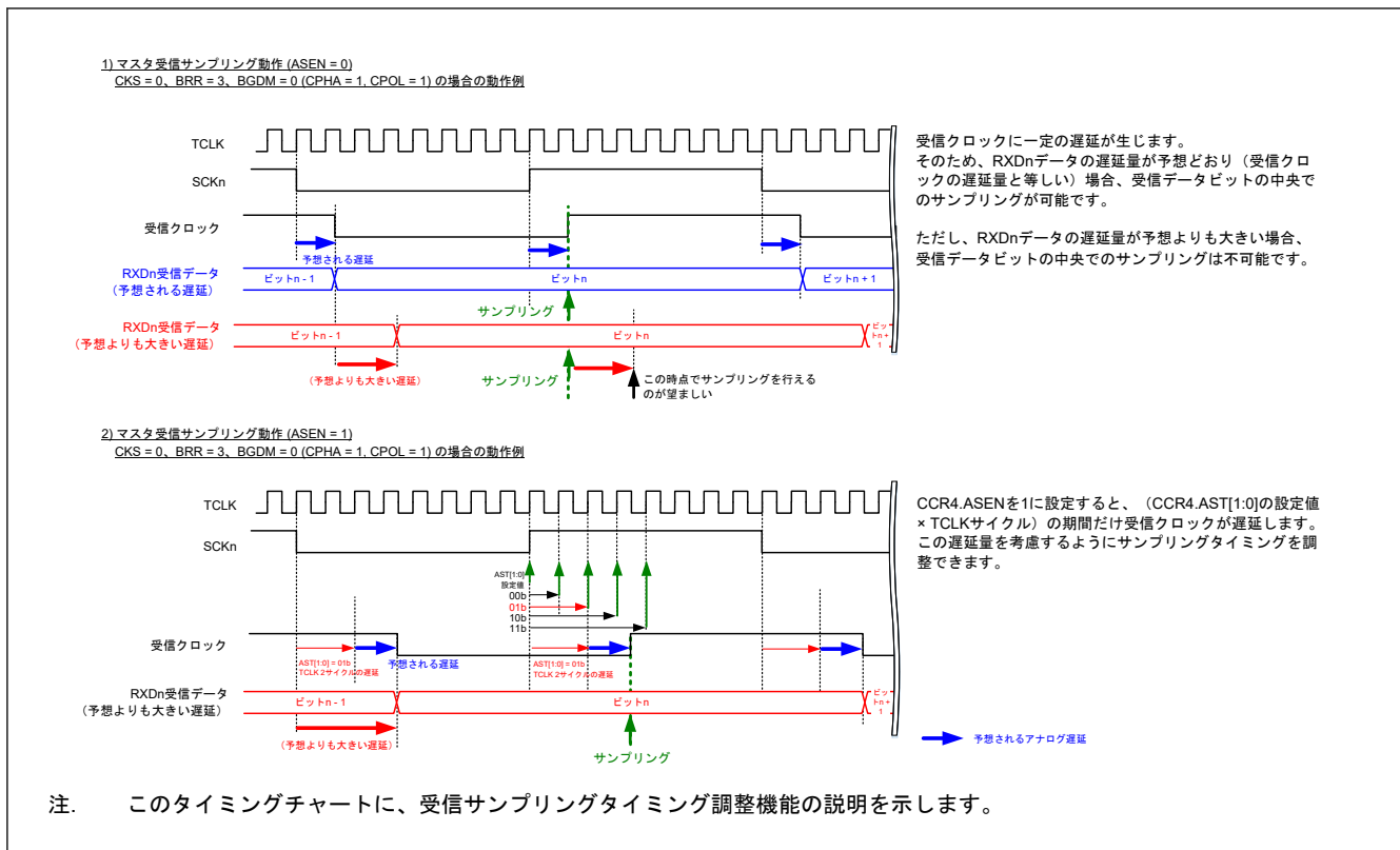
図 30.73 クロック同期式モード（マスタ）での受信サンプリングタイミング調整動作
