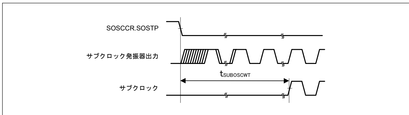
図 52.19 サブクロック発振開始タイミング
