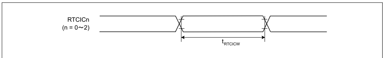
図 52.28 RTCICn 入力タイミング
