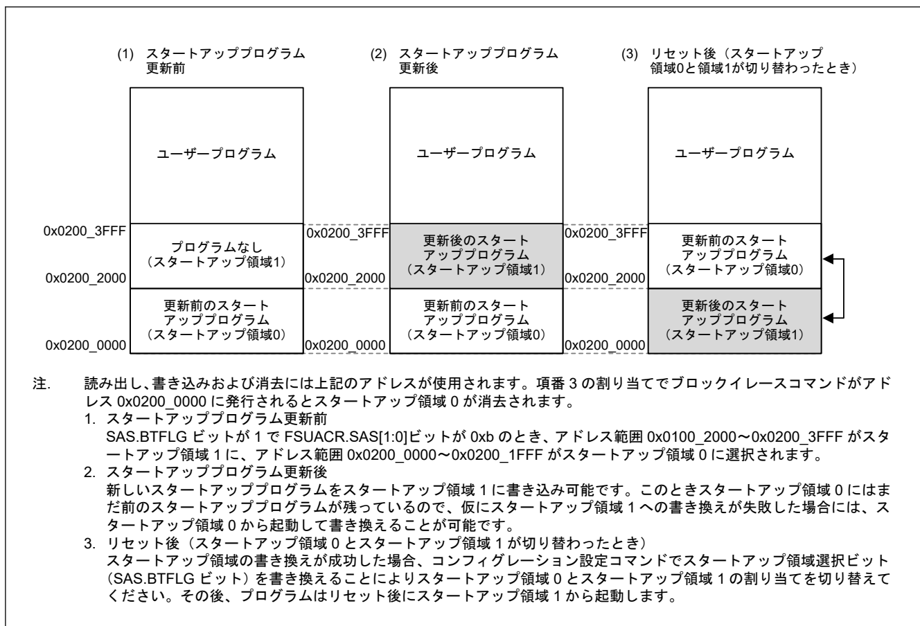
図 49.29 スタートアッププログラムプロテクションの概念 (セキュアエイリアスの場合)
