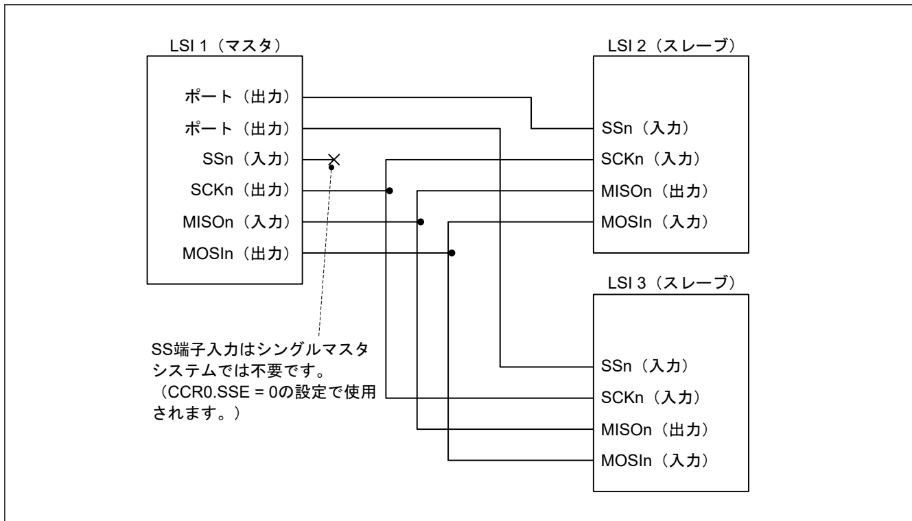
図 30.98 簡易 SPI モードでの接続例 (シングルマスタ時、CCR0.SSE ビット = 0)
