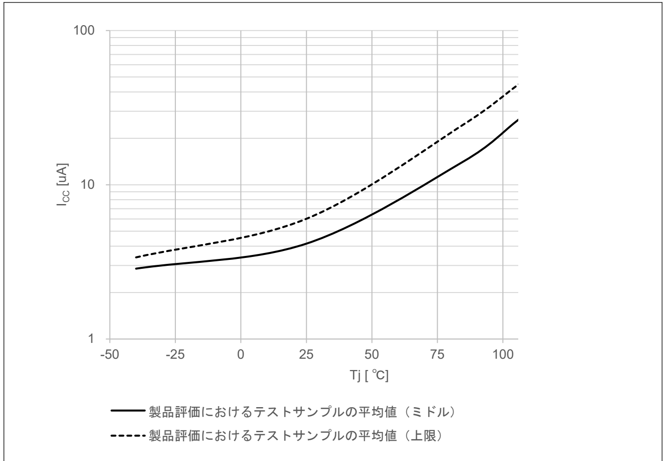
図 52.5 ディープソフトウェアスタンバイモード1における温度依存性 (参考データ)
