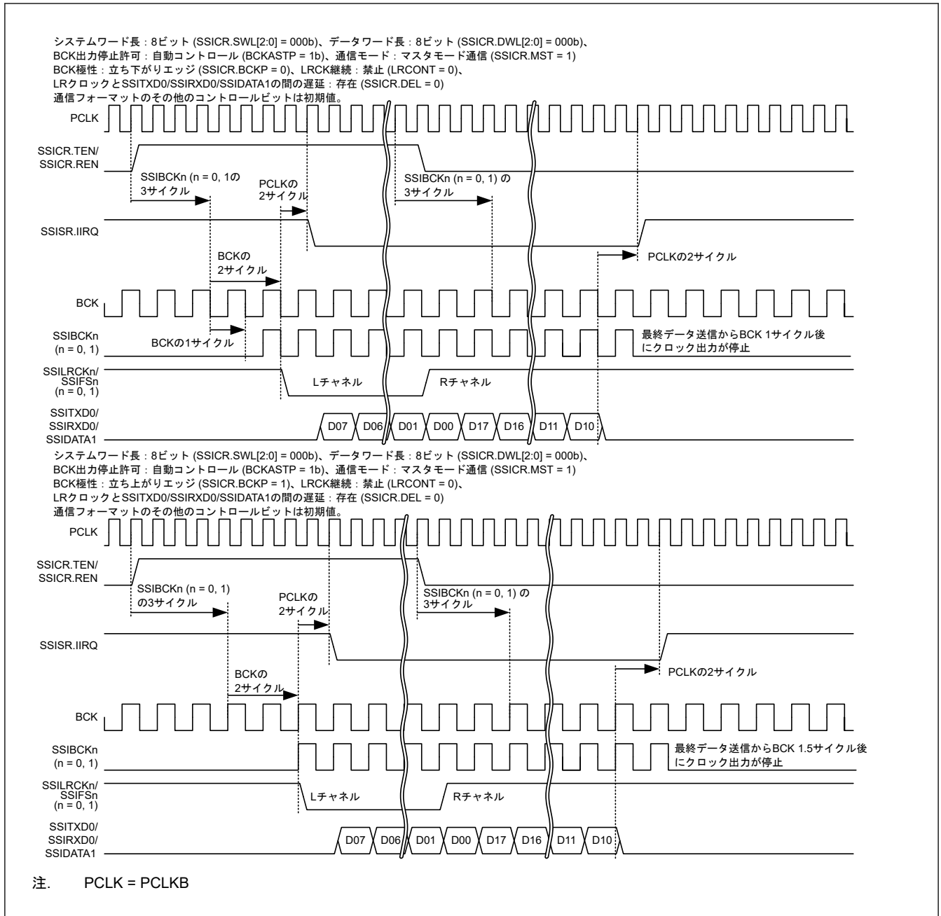
図 37.35 BCKASTP ビットの動作例 (BCKASTP = 1 での通信動作の場合)
