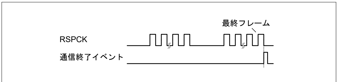
図 34.85 通信終了イベント出カタイミング (受信のみスレーブモード、クロック同期式動作)
