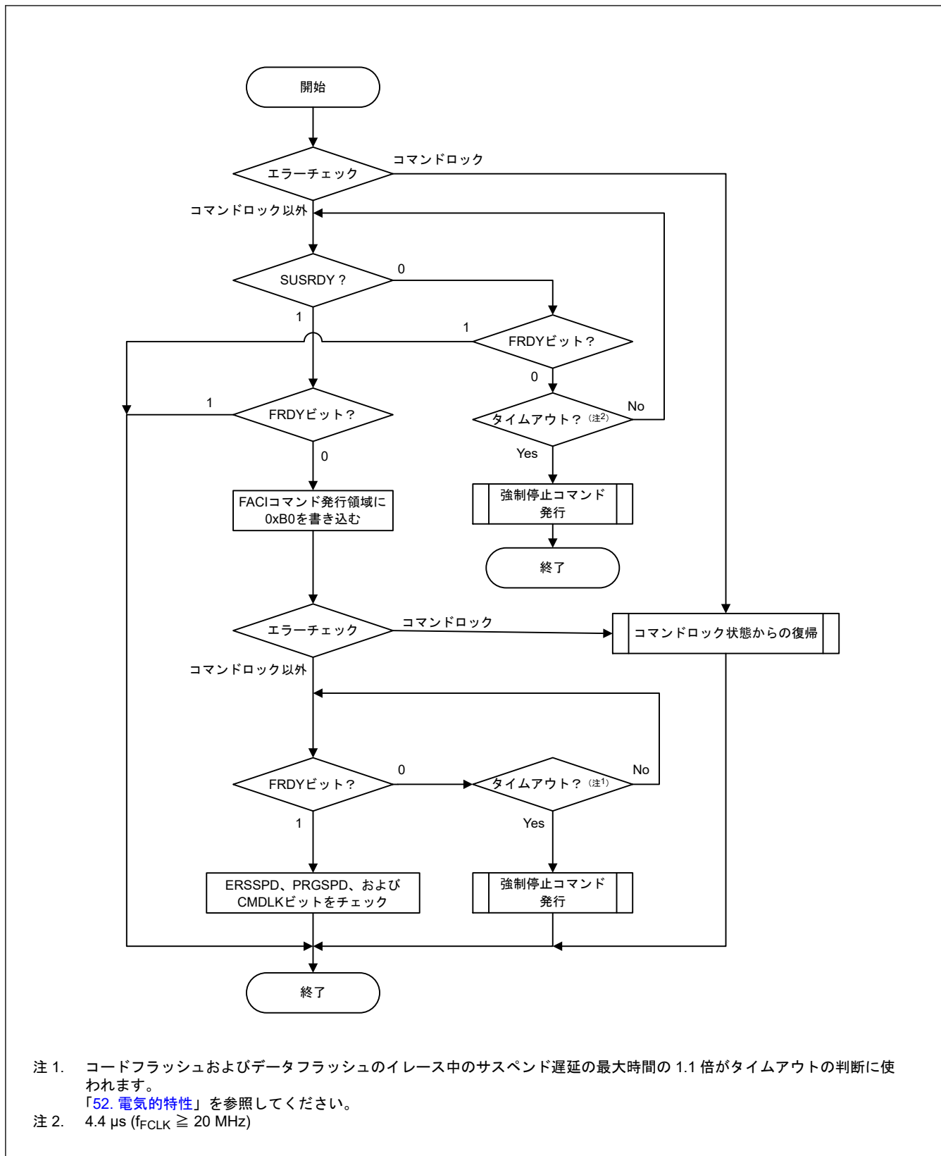
図 49.17 P/E サスペンドコマンドの使用フロー
