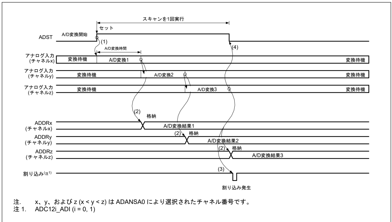
図 42.8 シングルスキャンモードの基本動作例（アナログ入力（チャンネル x~z）選択）
