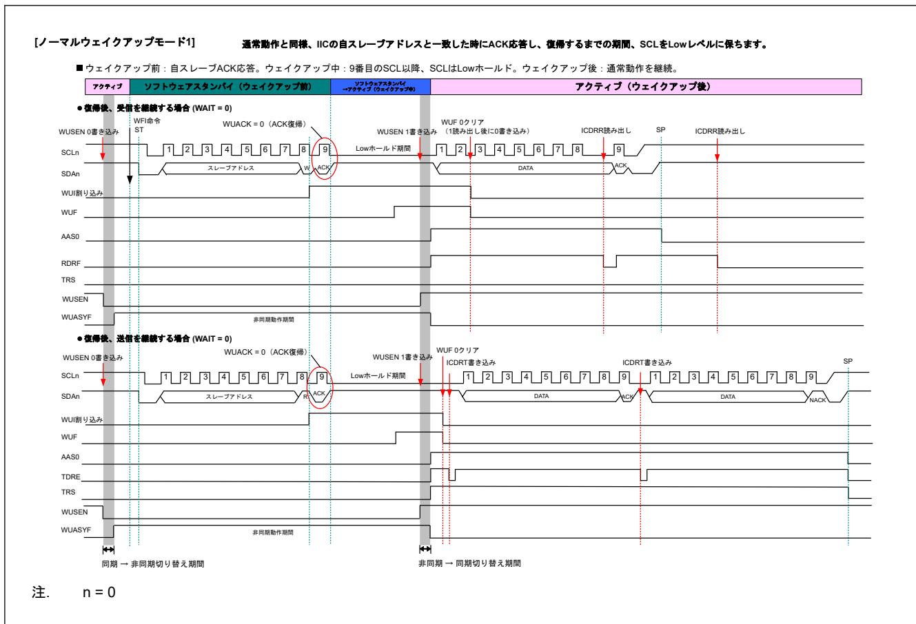
図 31.32 ノーマルウェイクアップモード1のタイミング
