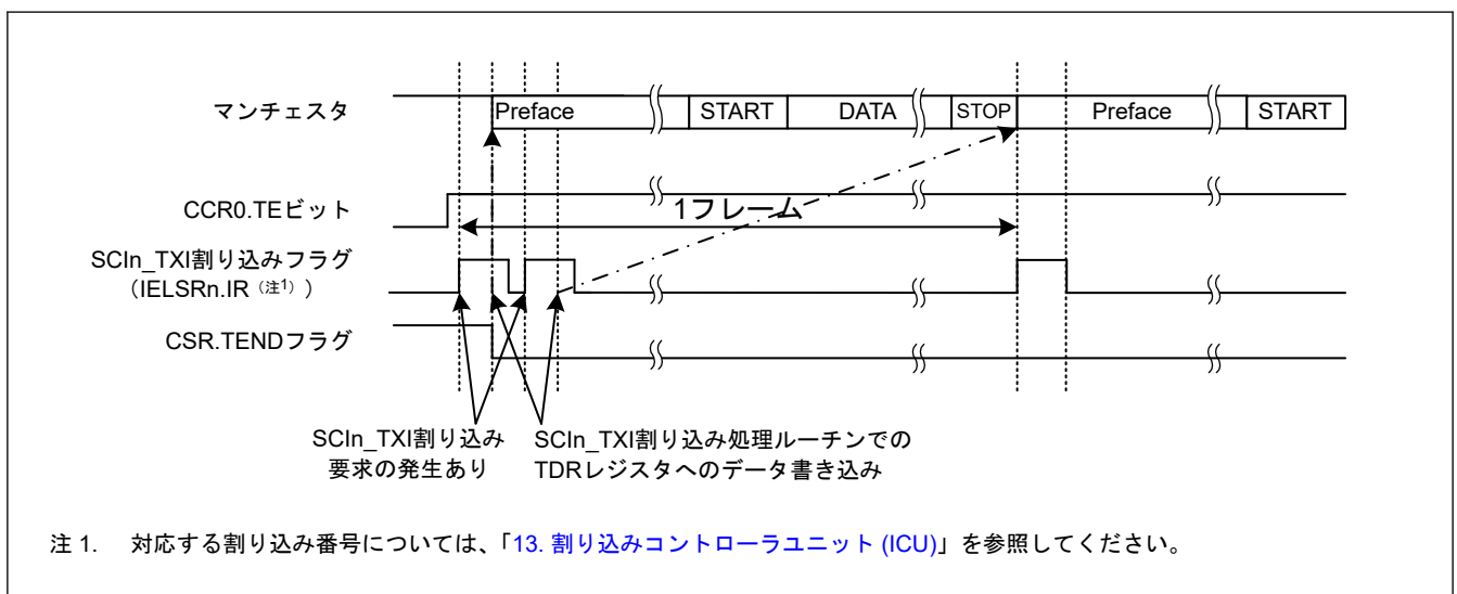
図 30.52 マンチェスタモードにおけるシリアル送信の送信開始動作の例 (プレフィスあり、CTS 機能なし)
