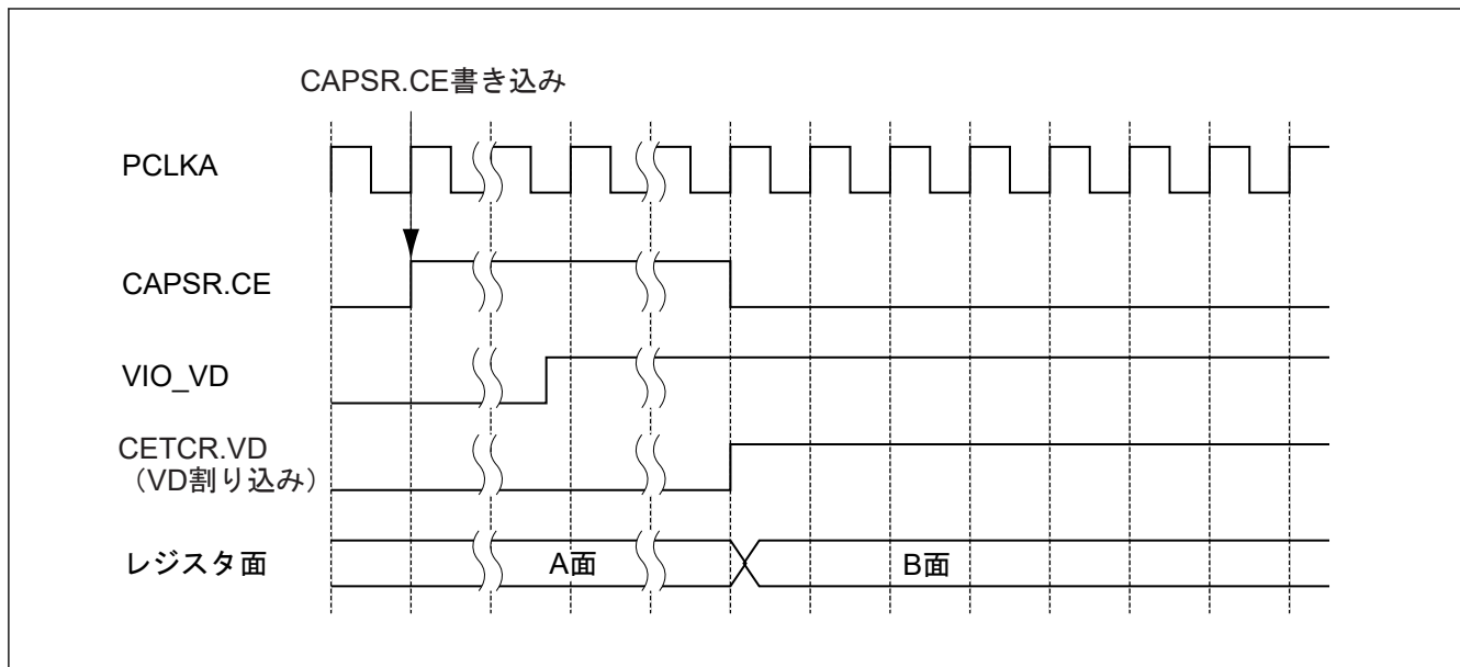
図 50.2 レジスタ面切り替えタイミング (データイネーブル取り込みモードかつ VD 正極性の場合)
