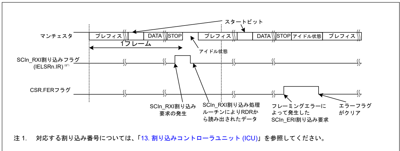
図 30.56 マンチェスタモードにおけるシリアルデータ受信の動作例（プレフィスあり）
