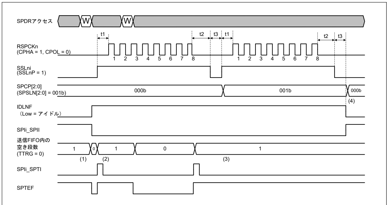
図 34.34 アイドル割り込み動作の例 (マスターモード/Motorola-SPI)
