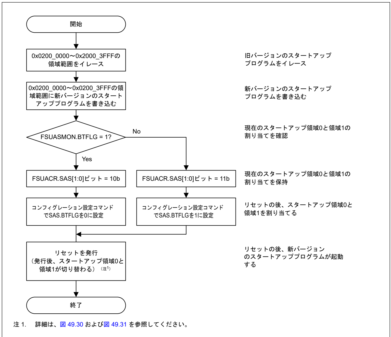
図 49.32 スタートアッププログラムプロテクションの概念 (セキュアエイリアスの場合)
