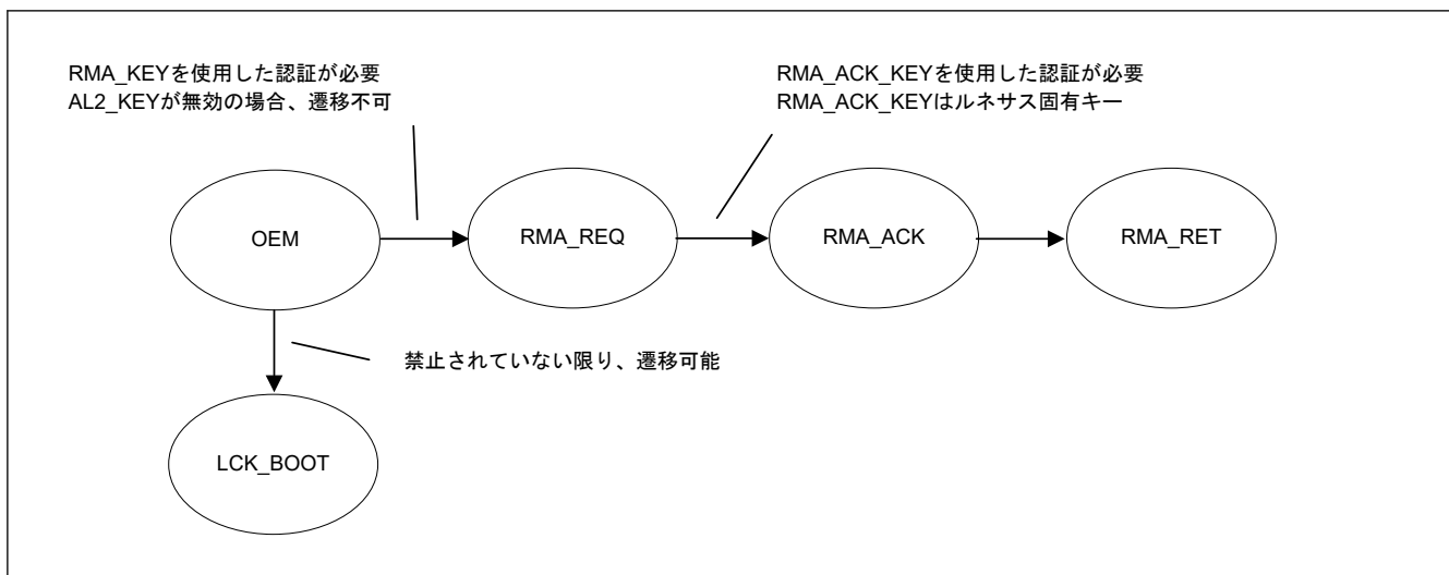
図 40.7 デバイスライフサイクル状態
