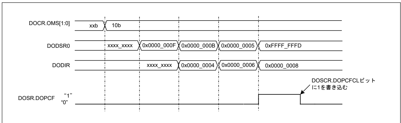
図 46.9 データ減算モードの動作例
