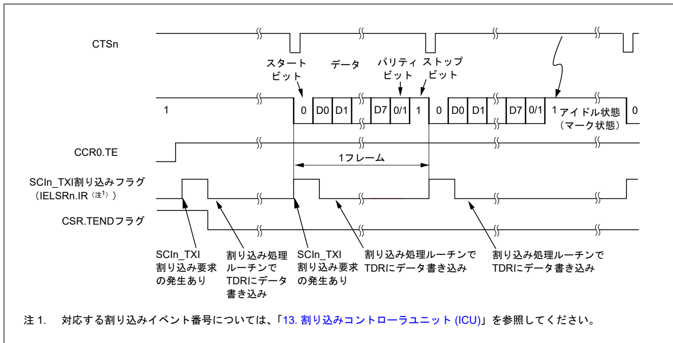
図 30.13 調歩同期式モードにおけるシリアル送信の動作例 (2) (8 ビットデータ/パリティあり/1ストップビット/CTS 機能使用/送信開始時)
