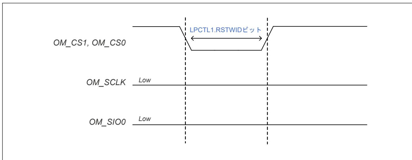
図 35.21 CS のみパターン
