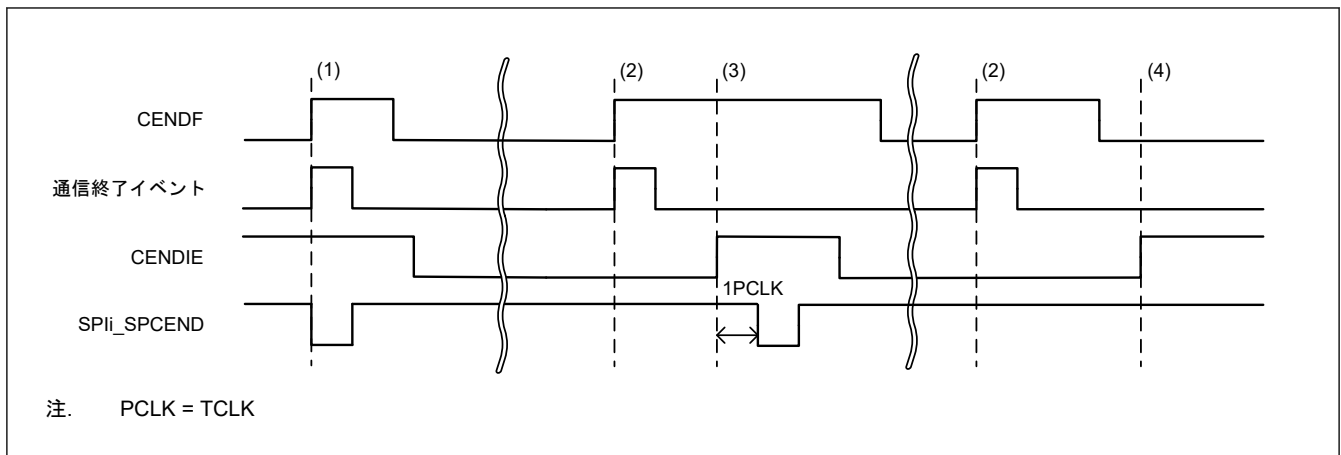
図 34.46 通信終了割り込みの動作例 (イネーブル制御)
