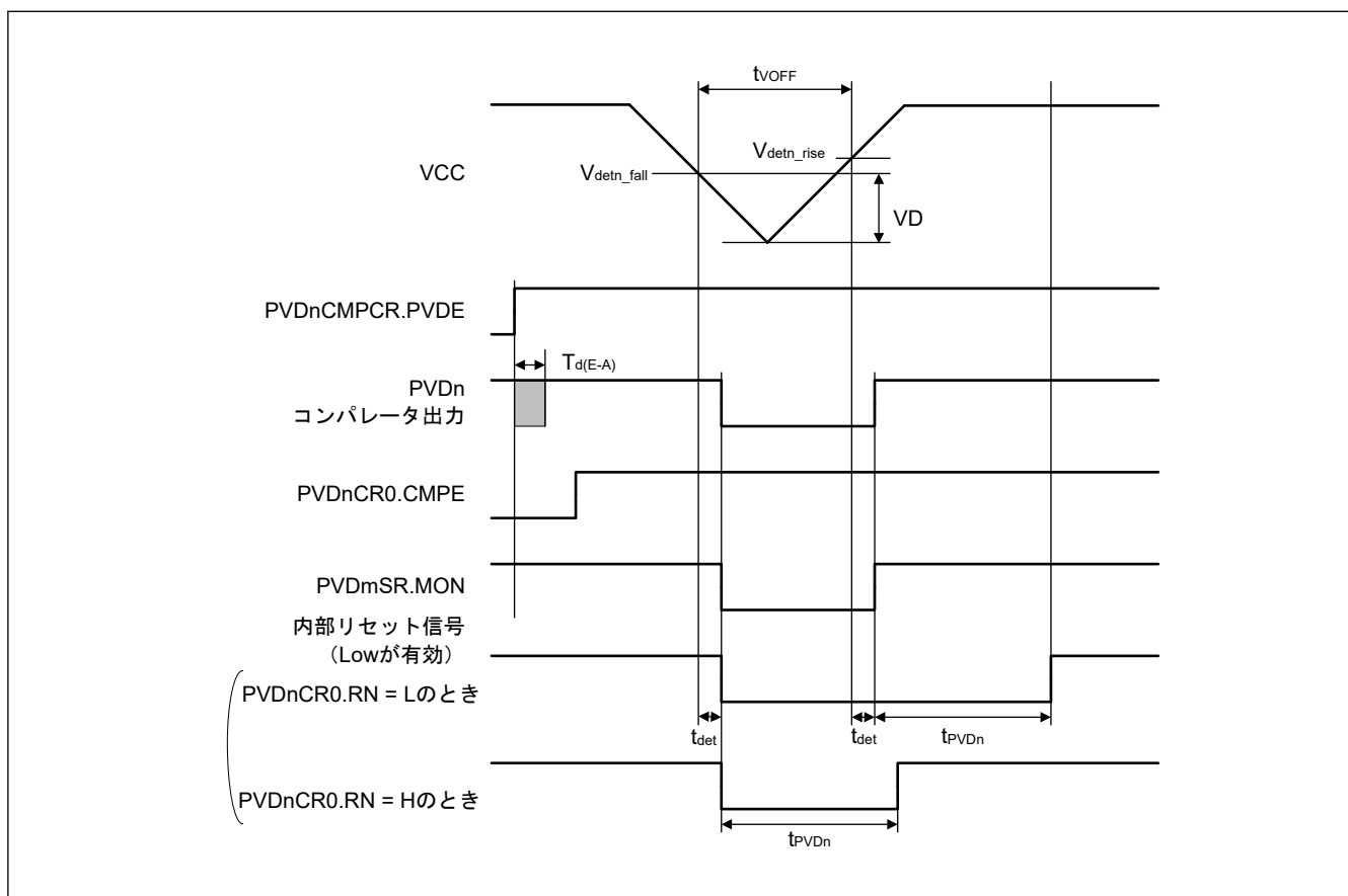
図 52.82 電圧検出回路タイミング ( V_{detn} ) ( n = 1, 2 )
