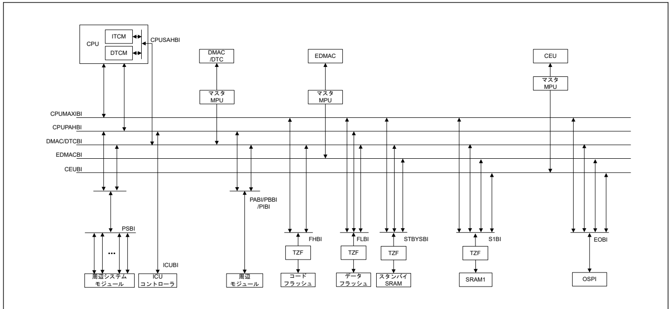
図 14.1 システムバスの接続
