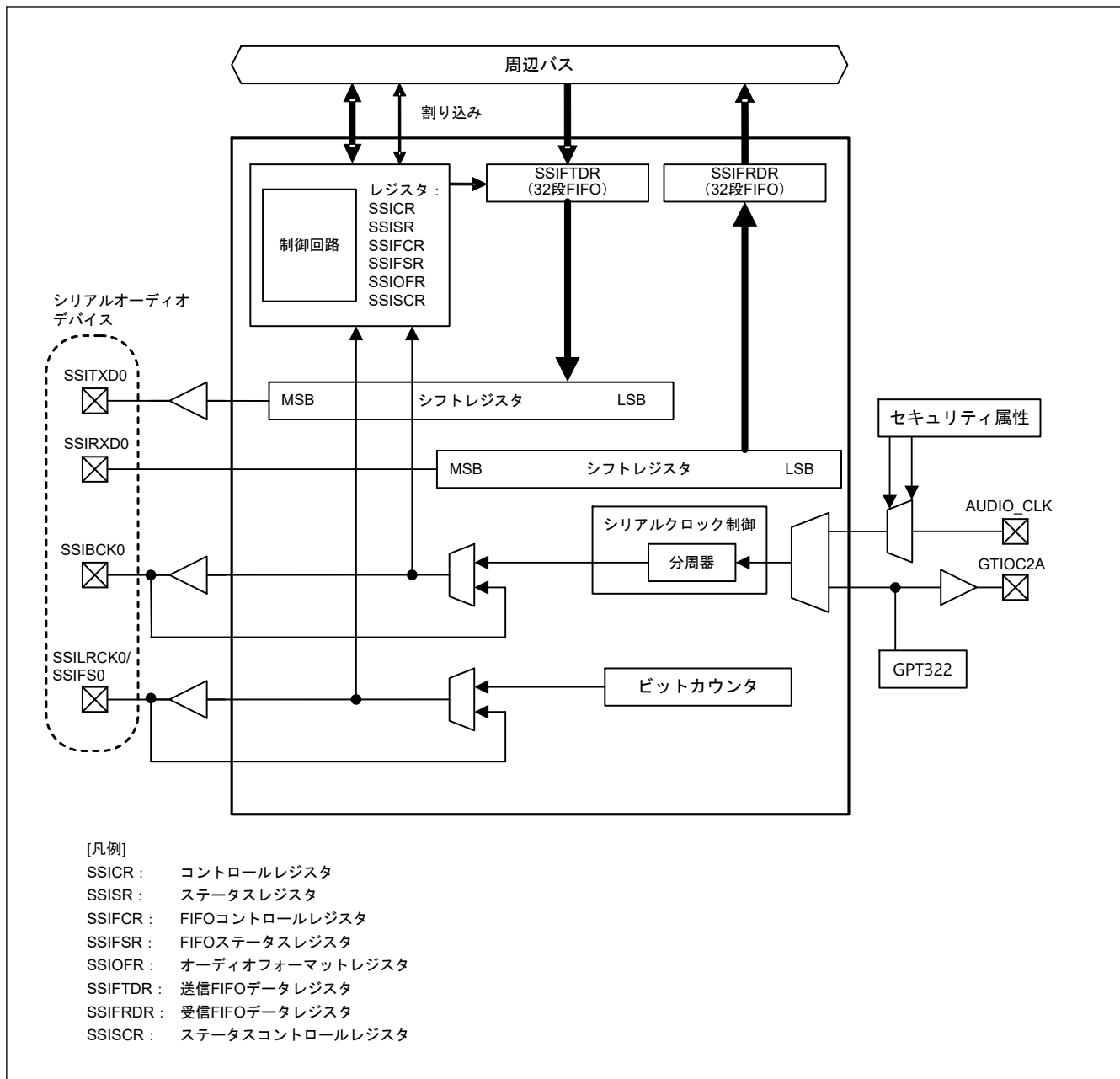
図 37.2 SSIE ブロック図 (SSIE0)
