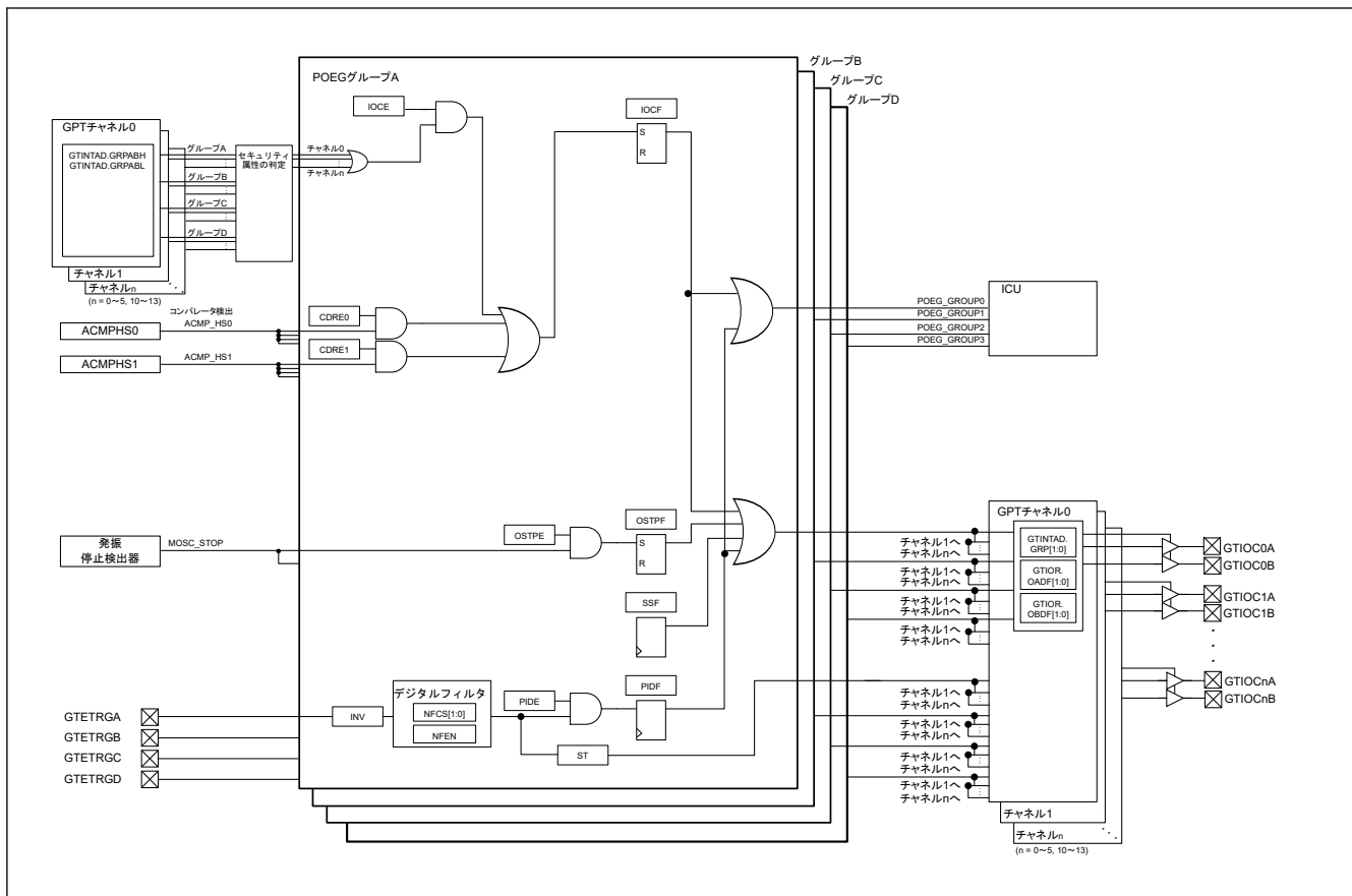
図 20.1 POEG ブロック図
