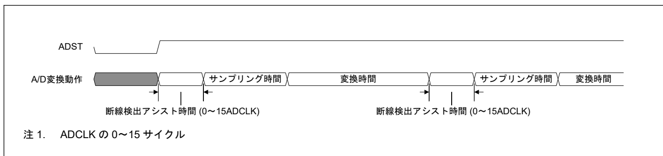
図 42.38 断線検出アシスト機能を使用した場合の A/D 変換動作図
