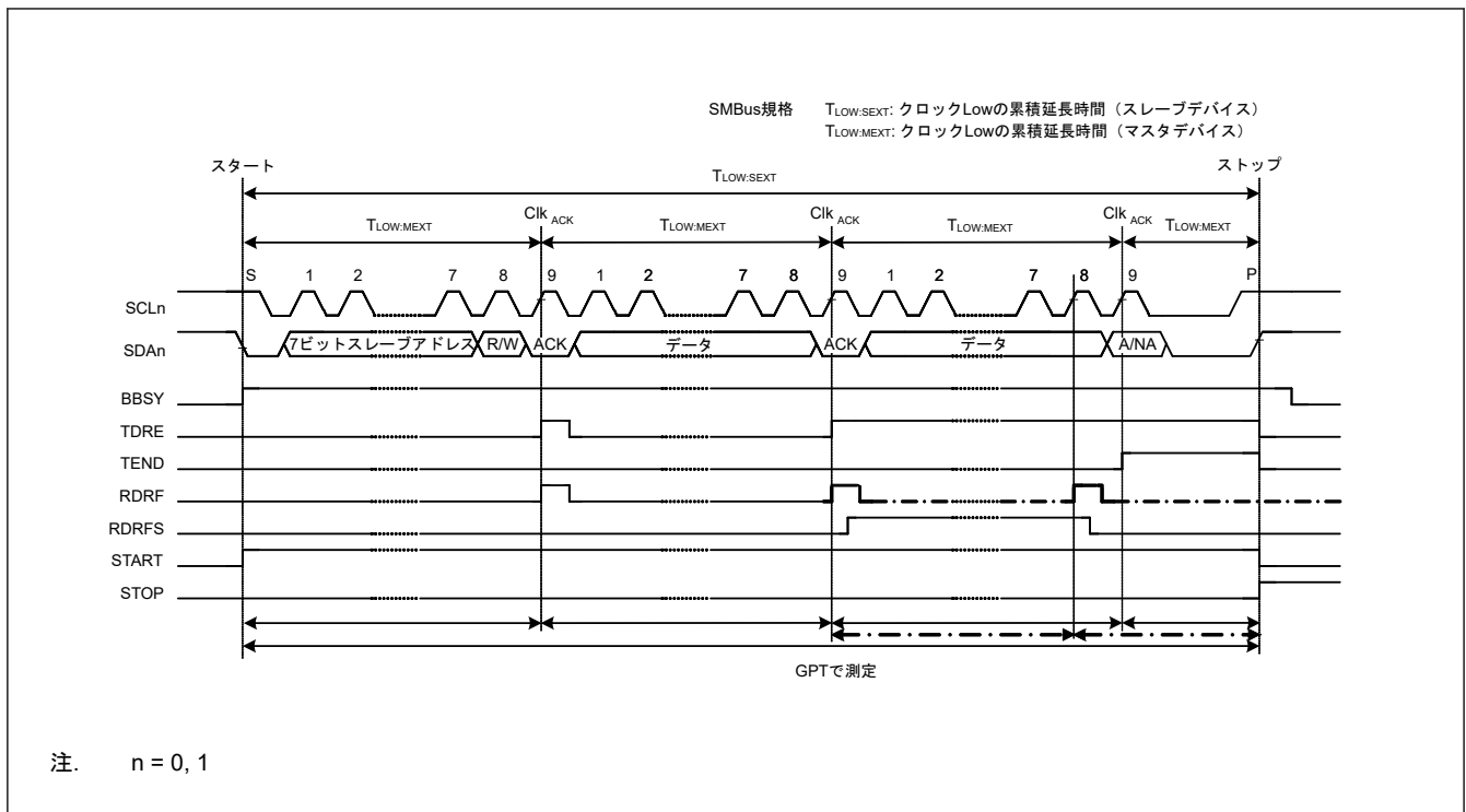
図 31.50 SMBus タイムアウト測定
