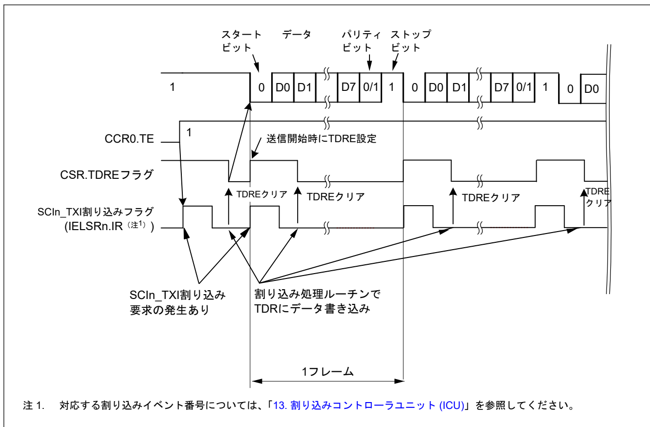
図 30.15 調歩同期式モードにおけるシリアル送信の動作例 (4) (8ビットデータ/パリティあり/1ストップビット/CTS 機能使用しない/送信途中~送信完了時)
