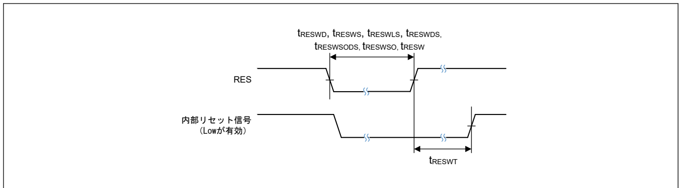
図 52.22 リセット入力タイミング
