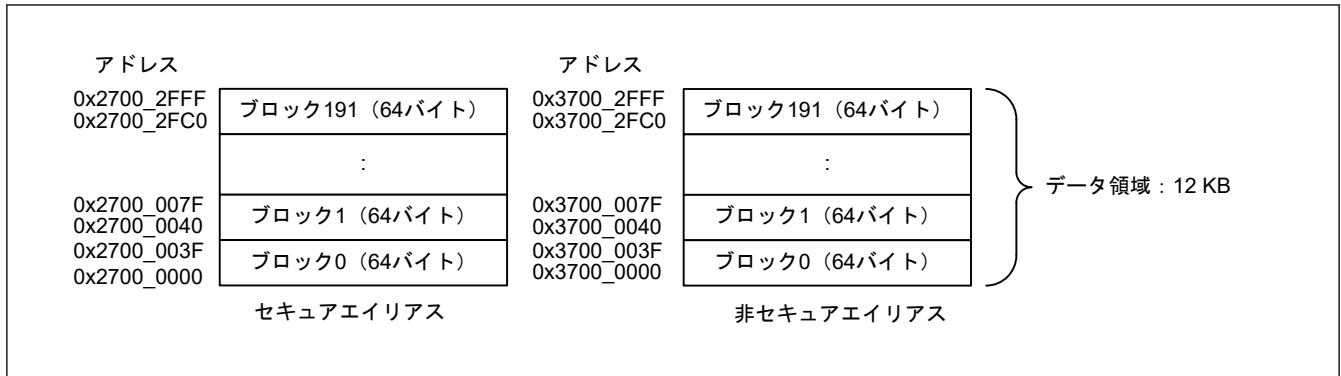
図 49.4 データフラッシュメモリのマップ
