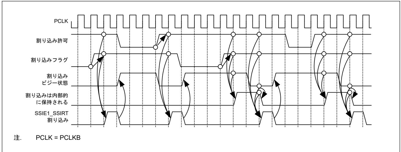
図 37.61 SSIE1_SSIRT 割り込みタイミング図
