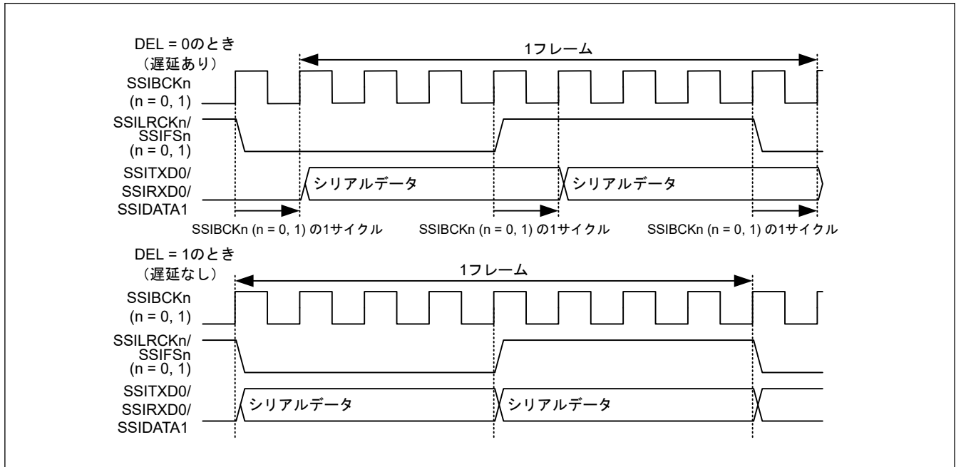
図 37.7 シリアルデータにおける遅延の設定
