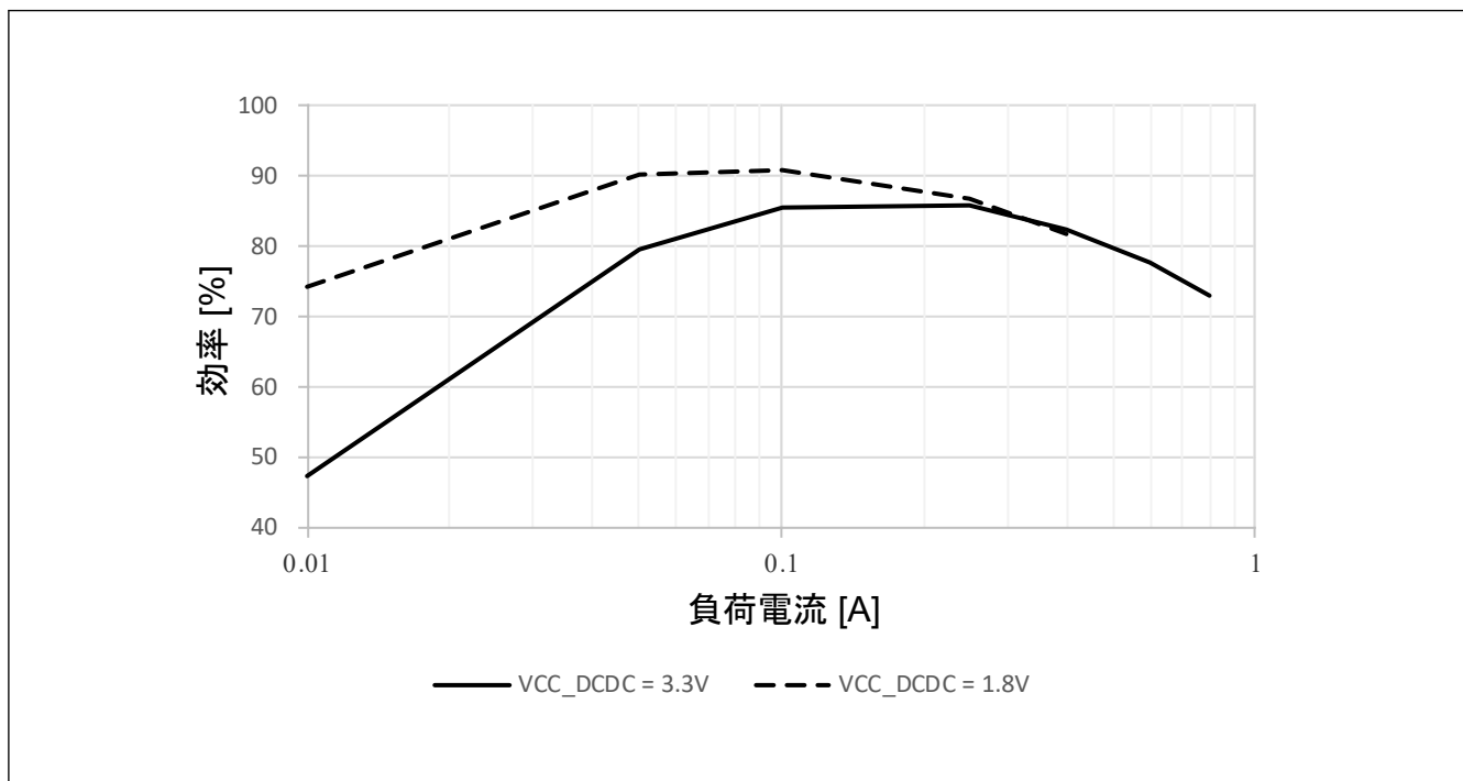
図 52.10 High-speed モード、 T_j = 105^\circ\text{C} における標準 DCDC 効率 (%) と負荷電流 (A)
