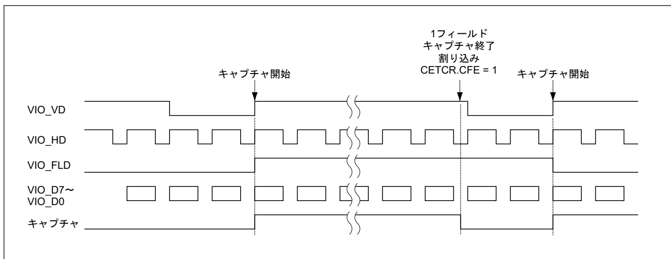
図 50.45 CFE 発生タイミング
