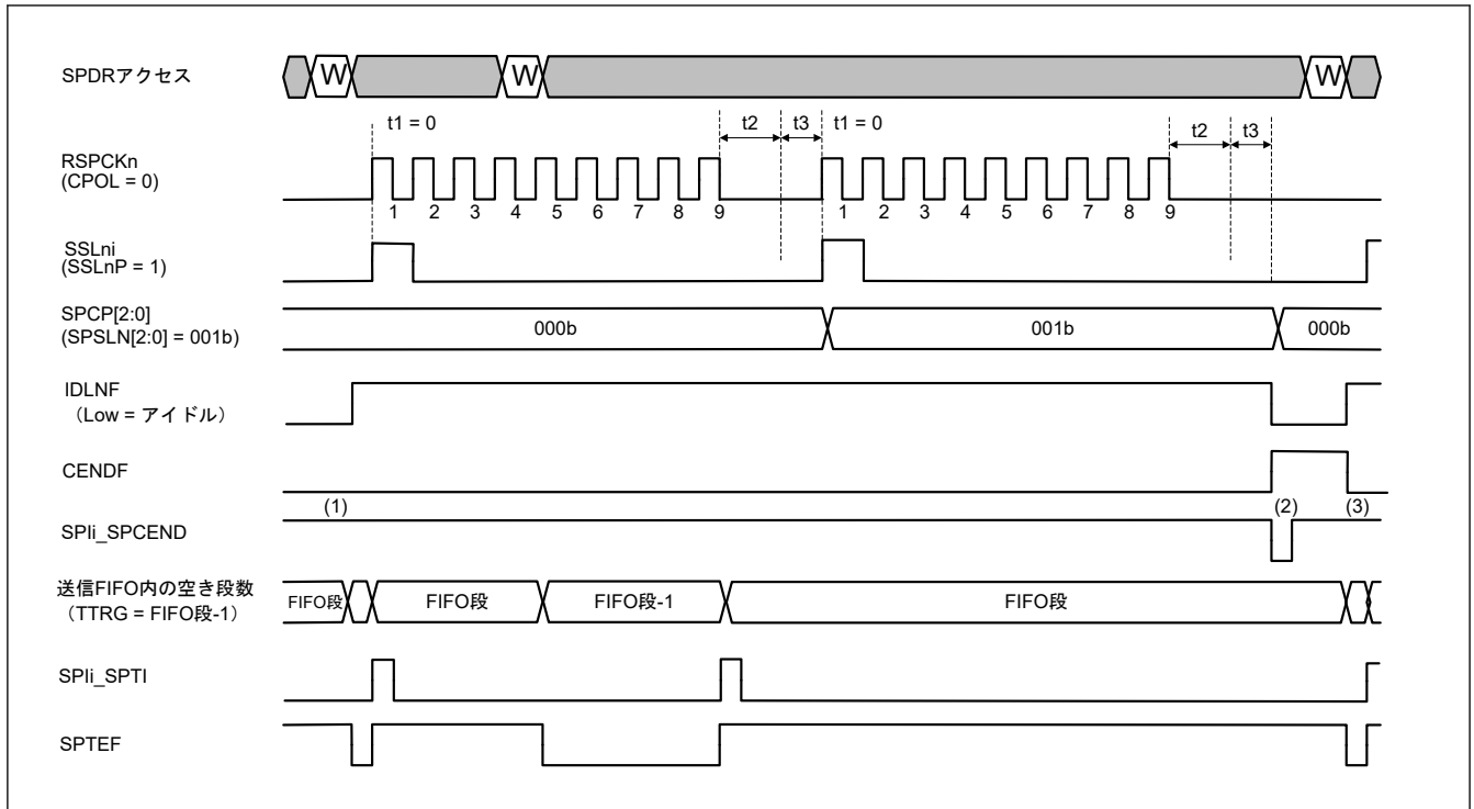
図 34.37 通信終了割り込み動作例（送受信/送信のみマスターモード/TI-SSP）
