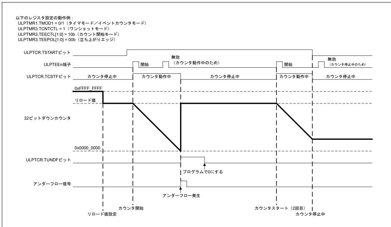
図 23.11 共通&amp;ワンショット&amp;カウンタ開始モードでの動作例
