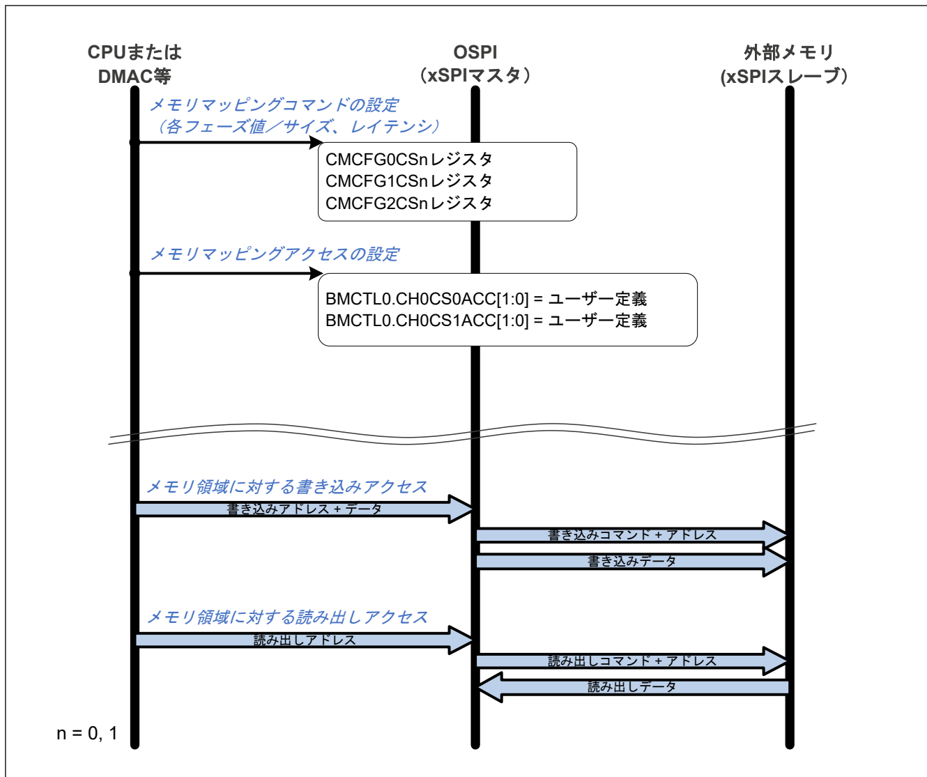
図 35.27 メモリマッピングのフロー
