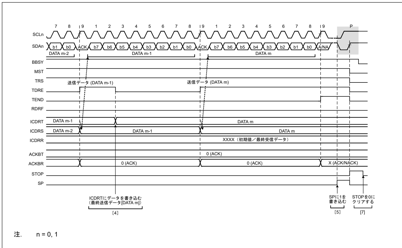
図 31.9 マスタ送信の動作タイミング (3)
