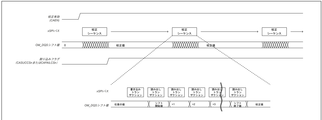
図 35.11 自動校正
