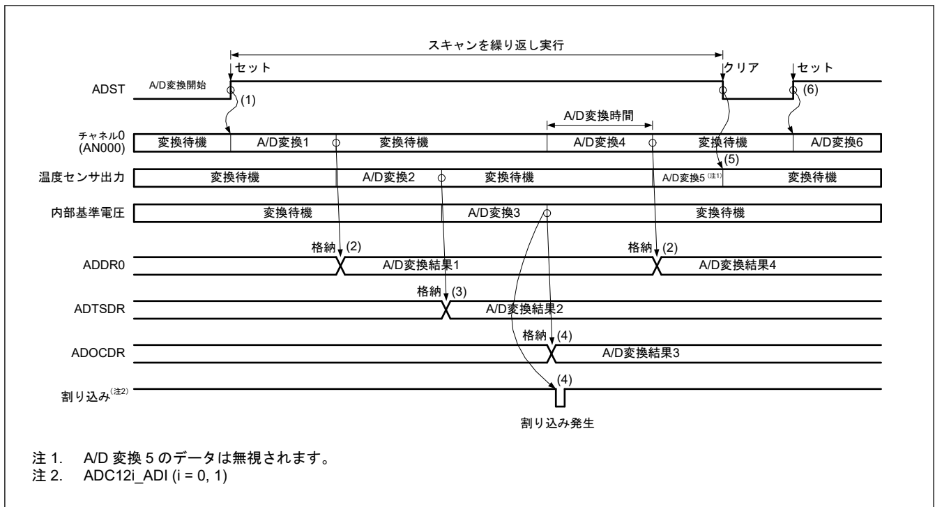
図 42.23 連続スキャンモードの基本動作例 (AN000、温度センサ出力または内部基準電圧選択)
