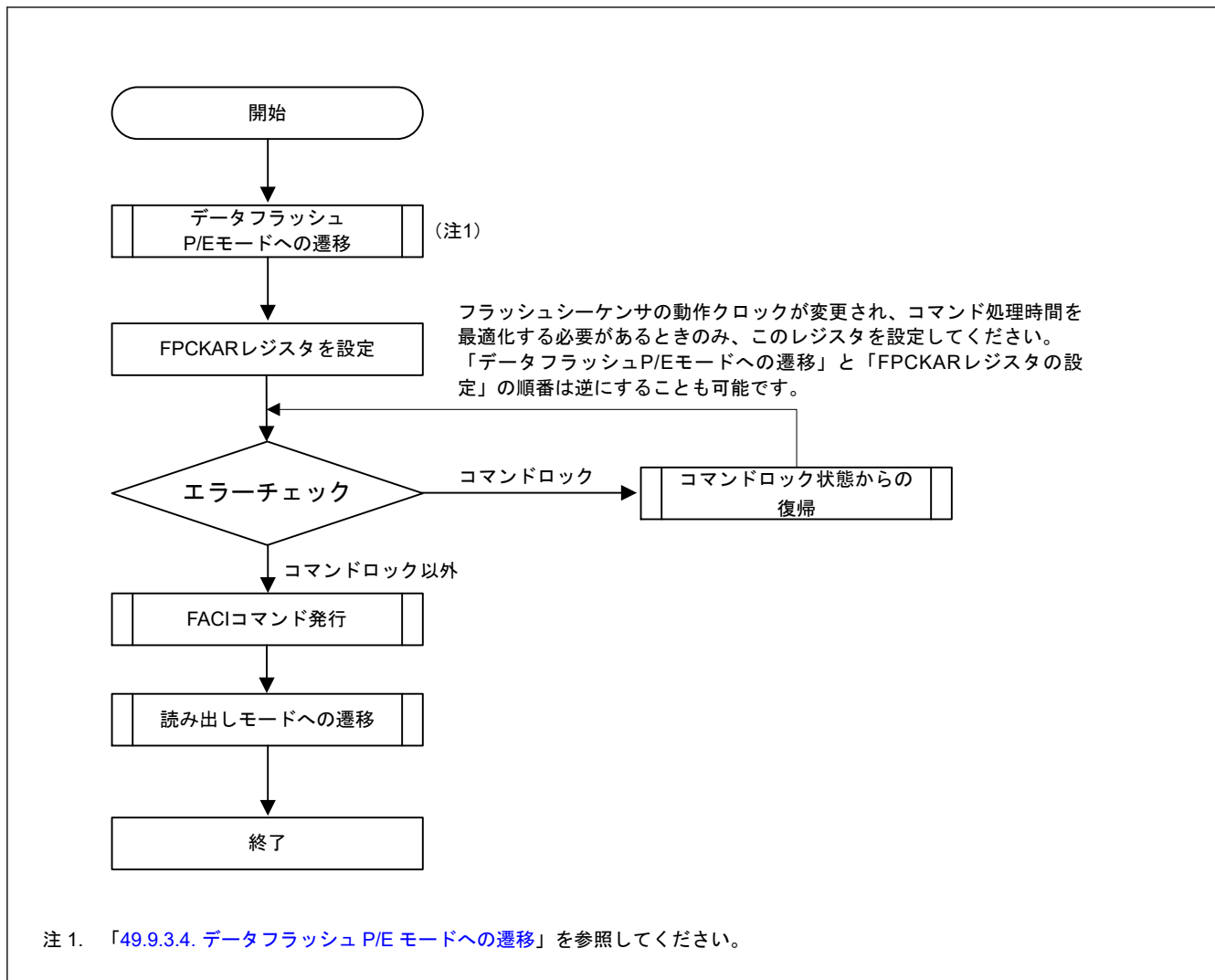
図 49.9 データフラッシュ P/E モードでのコマンド使用概要
