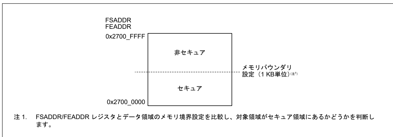
図 49.40 データ領域内のセキュア領域と非セキュア領域 (セキュアエイリアスの場合)
