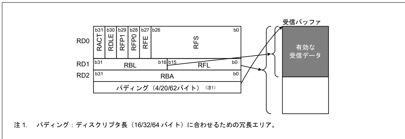
図 28.4 受信ディスクリプタと受信バッファの関係
