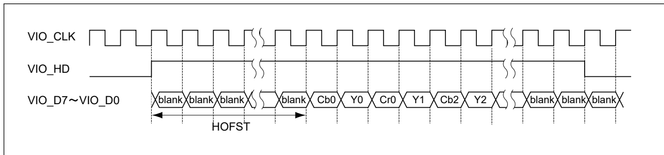
図 50.19 水平オフセット
