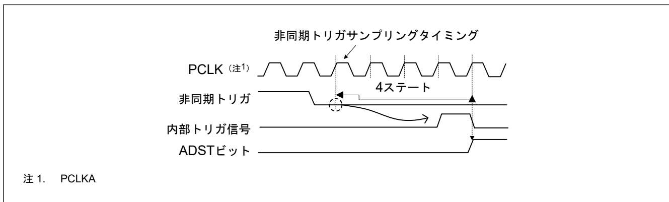
図 42.41 非同期トリガ入力タイミング
