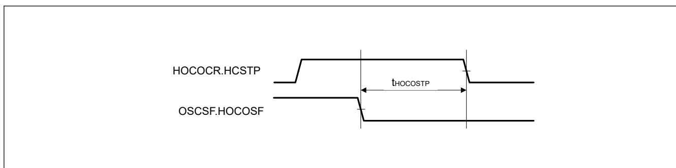
図 52.20 HOCO 停止幅時間
