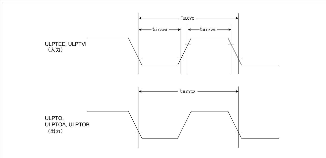
図 52.33 ULPT 入出力タイミング
