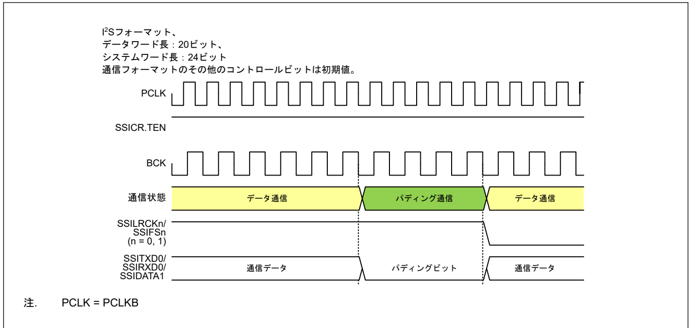
図 37.49 データ通信からパディング通信への遷移
