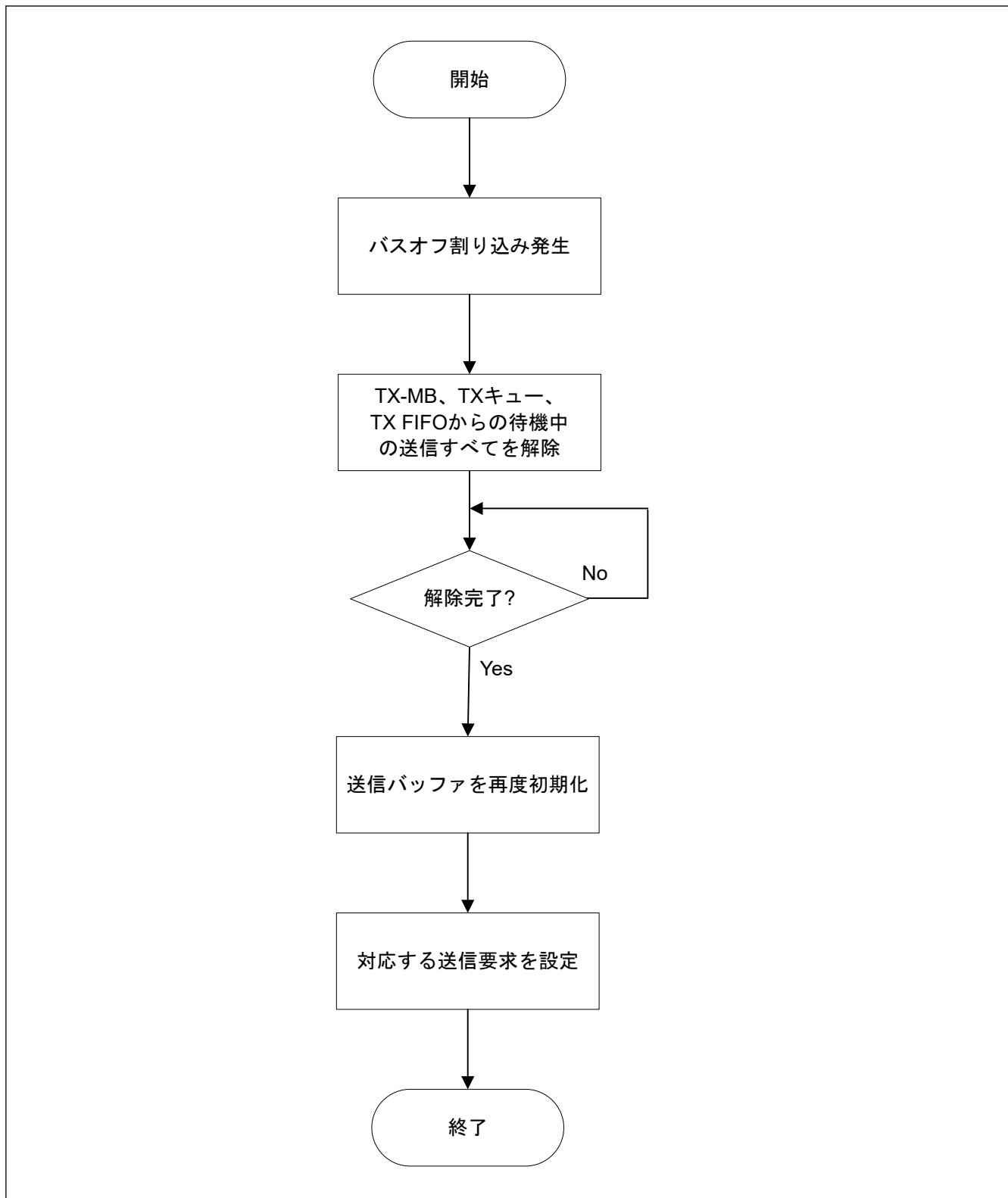
図 32.13 バスオフ中の送信の再初期化
