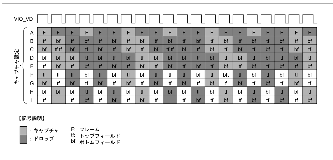
図 50.10 各キャプチャ設定におけるフレームドロップのタイミングイメージ (FDRP[7:0] = 0x2)
