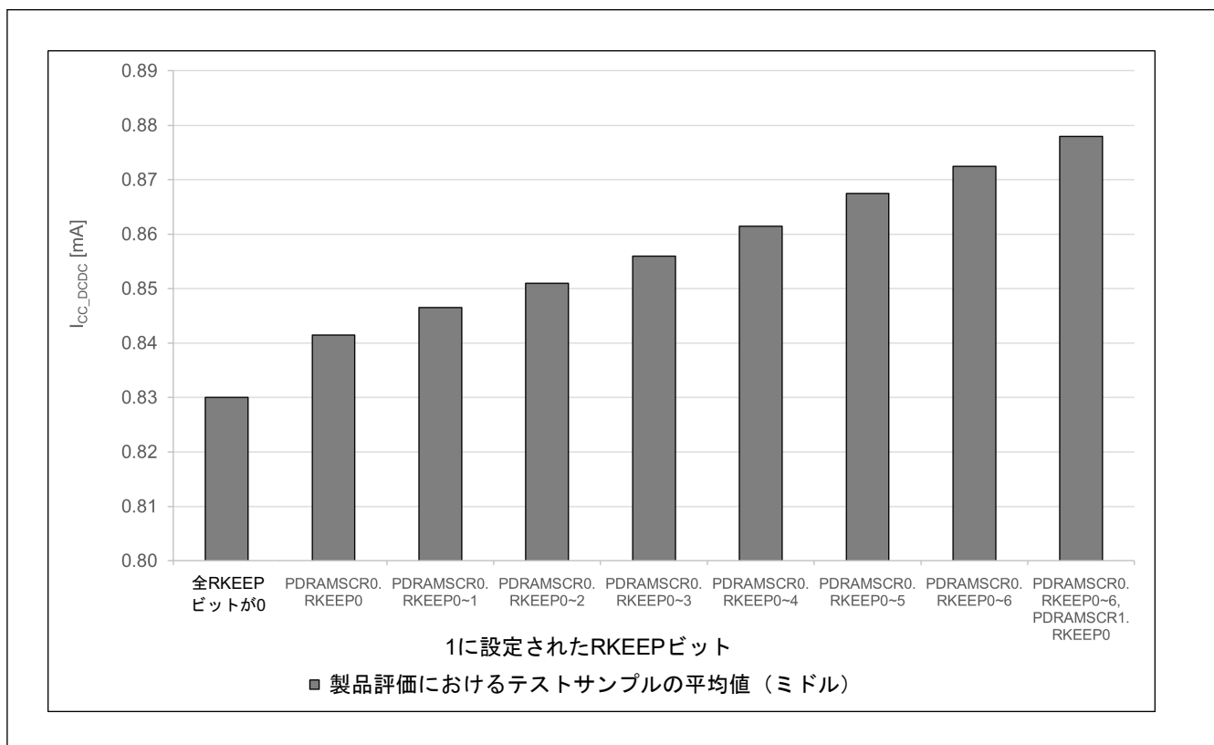
図 52.8 1 SRAM ステートあたりのソフトウェアスタンバイ電流 (参考データ)
