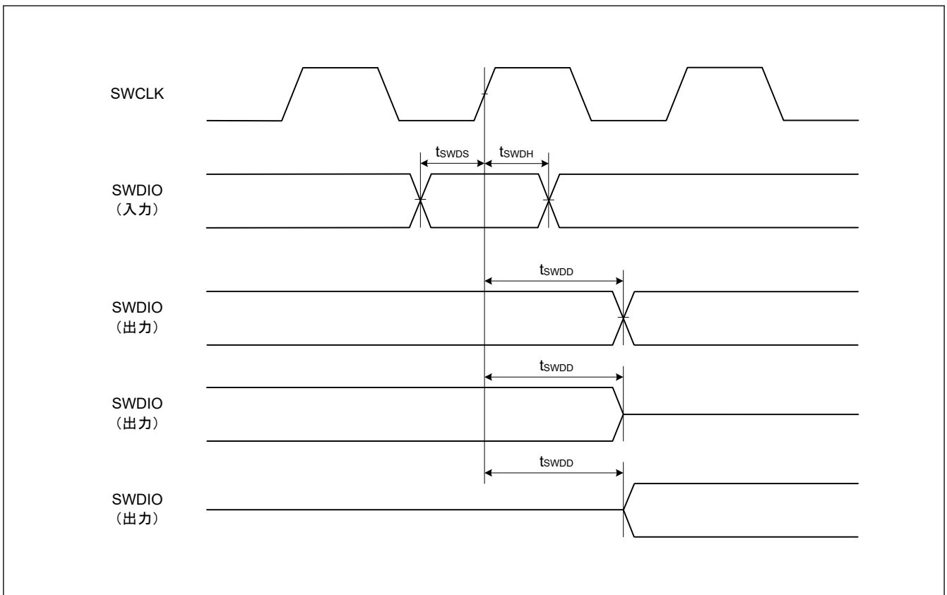
図 52.93 SWD 入出力タイミング
