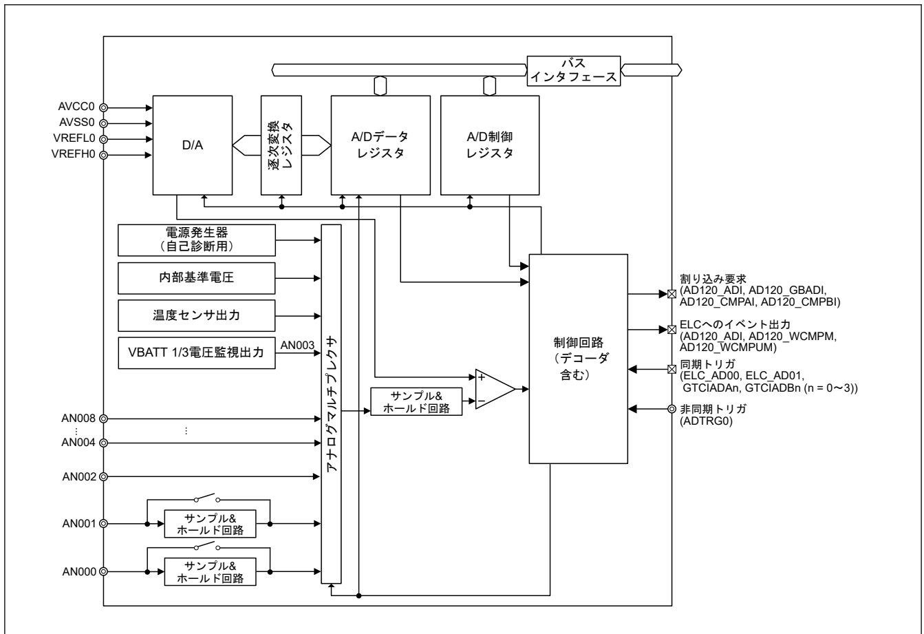
図 42.1 ADC12 のブロック図 (ユニット 0)
