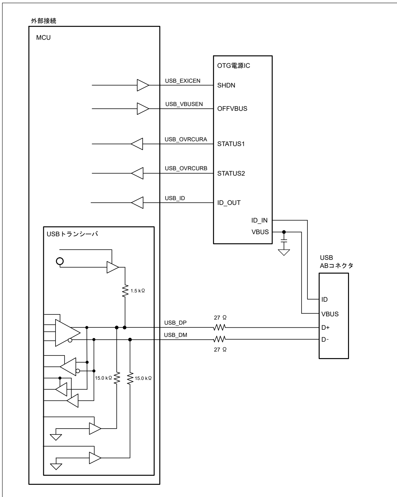
図 29.2 セルフパワーシステムでの OTG 接続例
