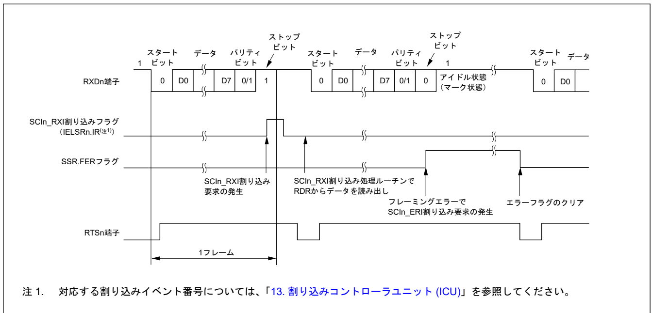
図 30.20 調歩同期式モードにおけるシリアル受信の動作例 (2) (RTS 機能を使用する場合) (8 ビットデータ / パリティあり / 1 ストップビットの場合)
