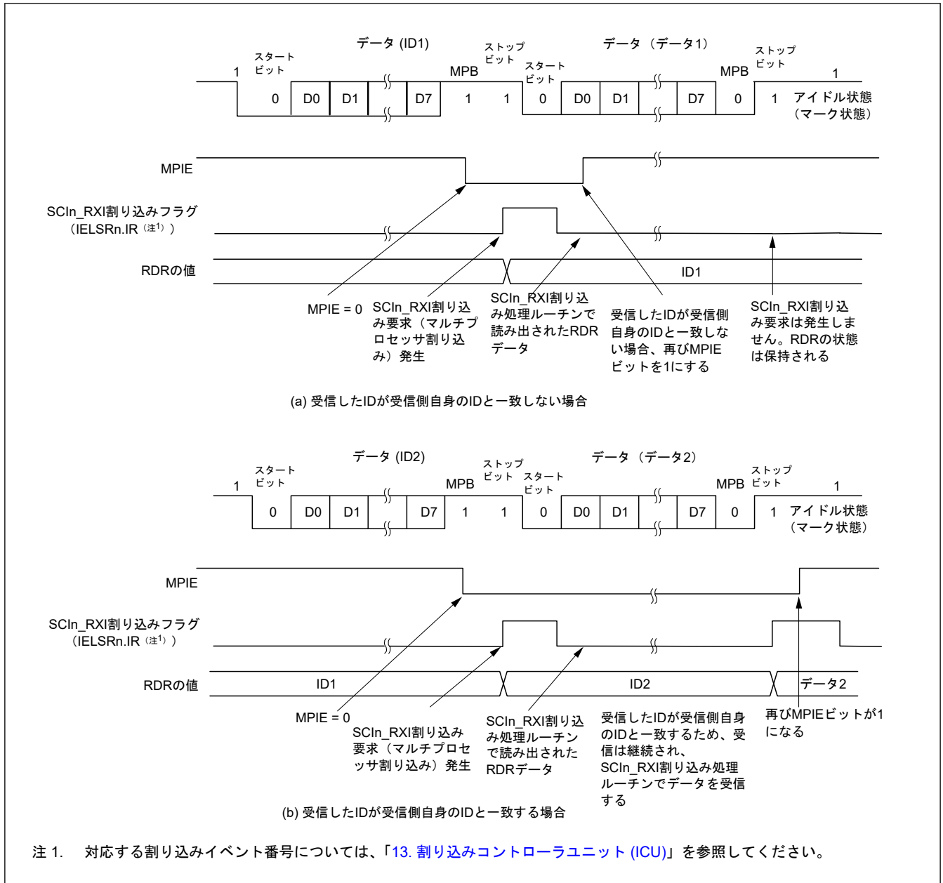
図 30.39 SCIの受信時の動作例 (8ビットデータ/マルチプロセッサビットあり/1ストップビットの場合)
