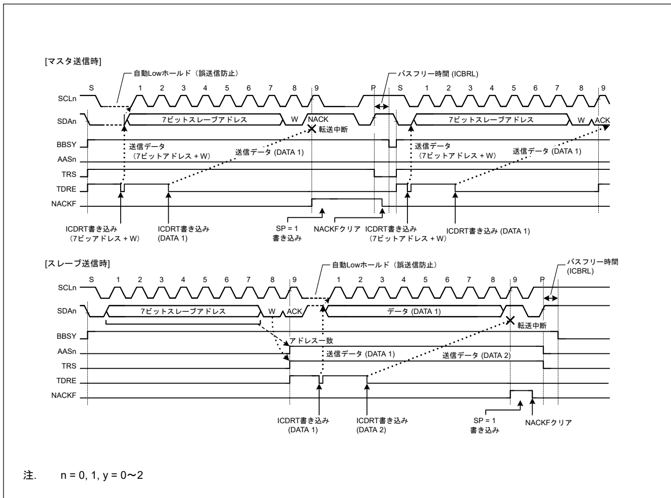
図 31.39 NACK 受信時のデータ転送中断動作 (NACK = 1 の場合)
