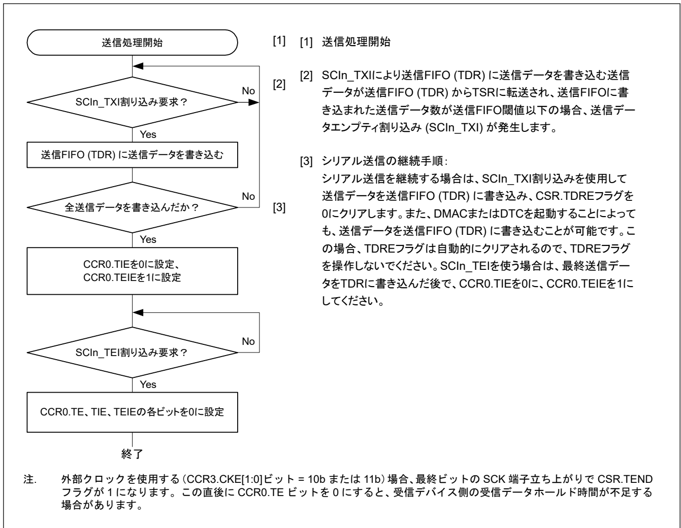
図 30.66 クロック同期式モードにおけるシリアル送信のフローチャート例 (FIFO 選択時)
