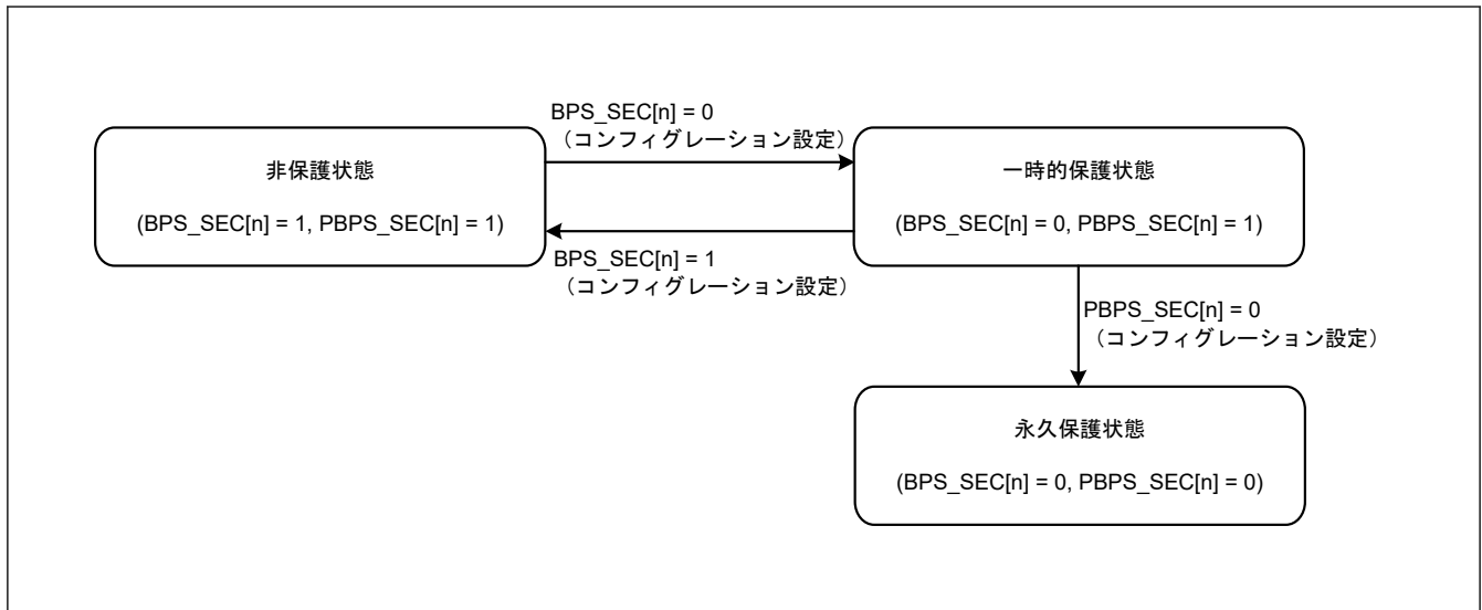
図 49.38 BPS_SEC[n]ビットおよびPBPS_SEC[n]ビットによるフラッシュシーケンサの状態遷移
