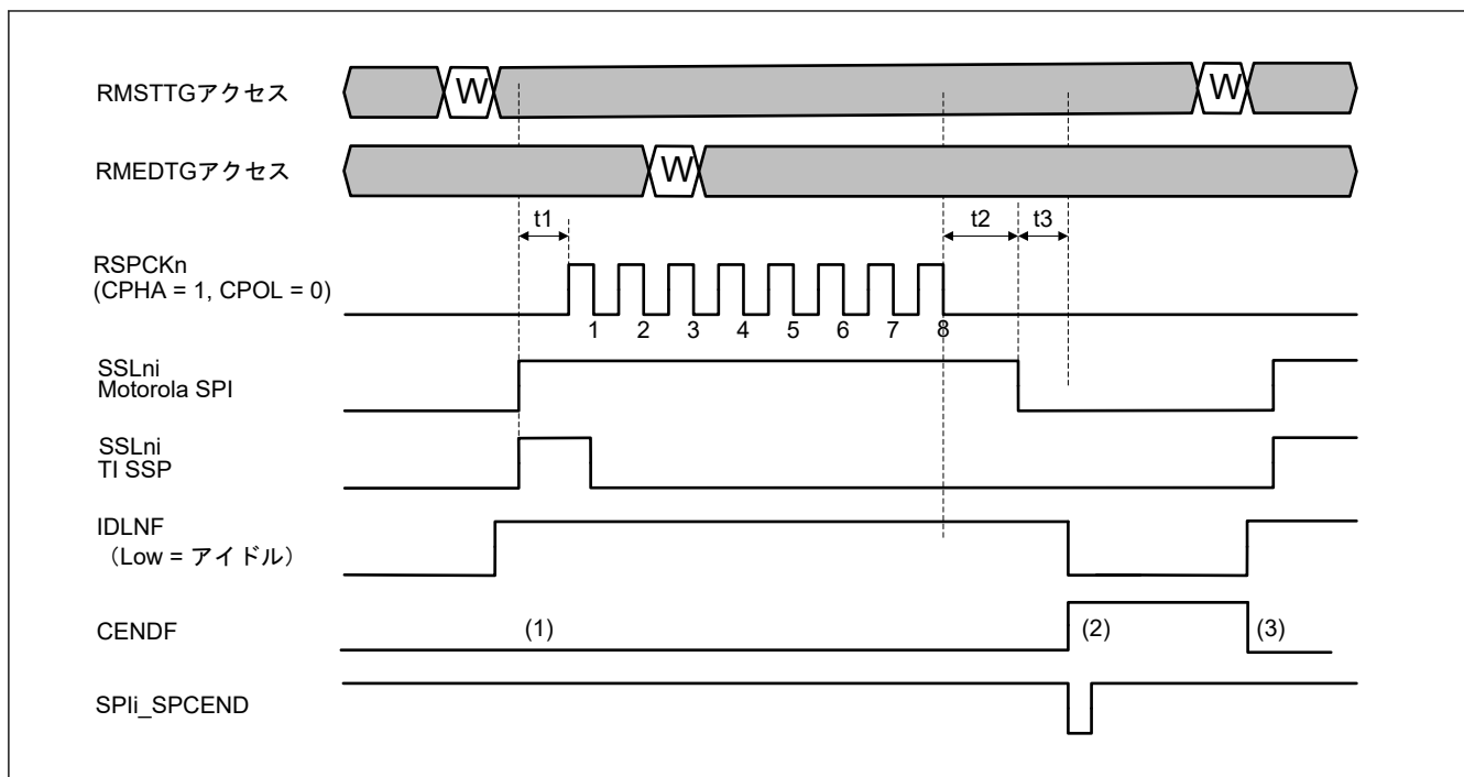
図 34.38 RMFM[4:0] = 0 時の通信終了割り込み動作例 (受信専用マスタモード/Motorola-SPI)
