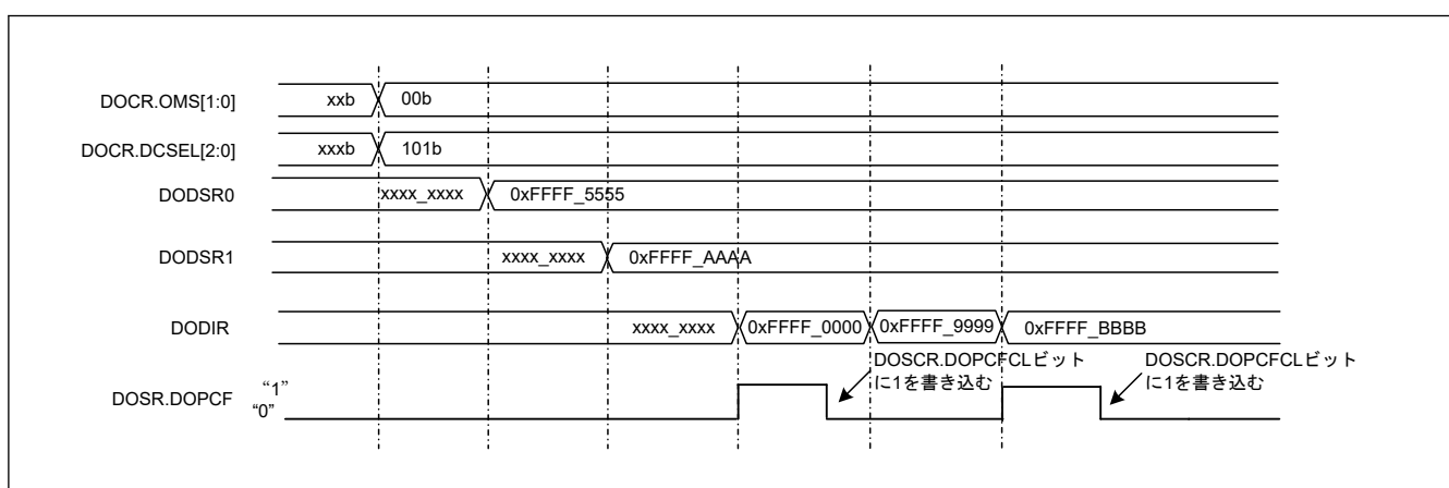
図 46.7 データ比較モードの動作例 (検出条件: ウィンドウの外側)
