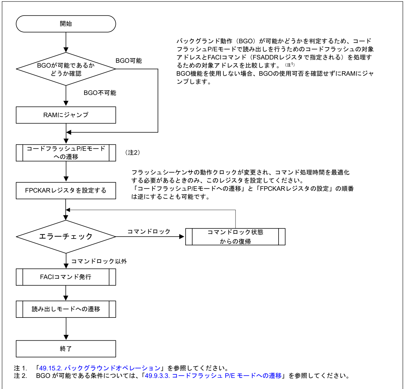
図 49.8 コードフラッシュ P/E モードでのコマンド使用概要
