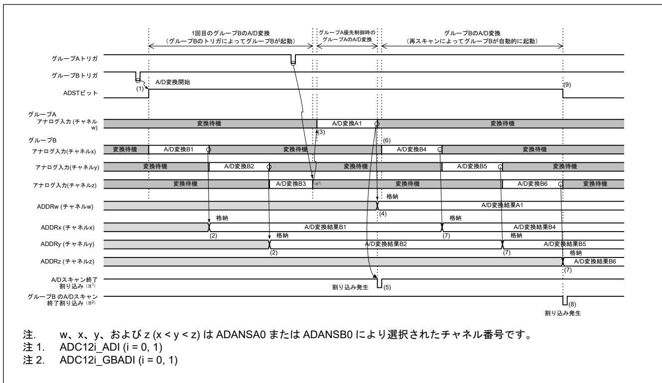
図 42.27 グループ優先動作の例 1-1: グループ B スキャン中のグループ A トリガ入力、再スキャンあり (ADGSPCR.GBRSCN = 1、ADGSPCR.GBRP = 0、および ADGSPCR.LGRRS = 0 の場合)
