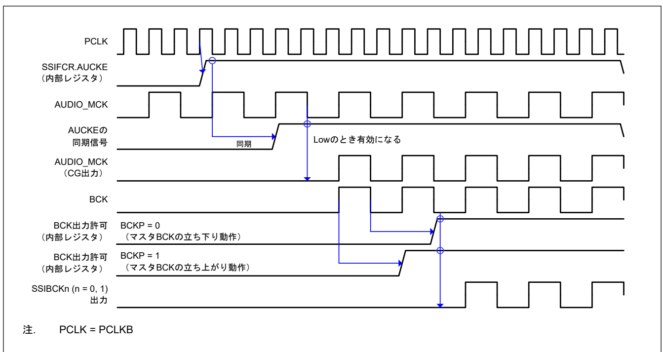
図 37.26 システムリセットからマスタモード通信開始までの動作のタイミング図
