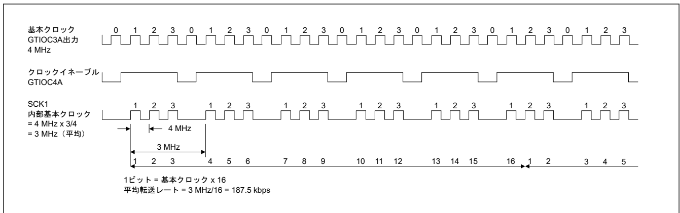
図 30.5 GPT クロック入力時の平均転送レート設定例
