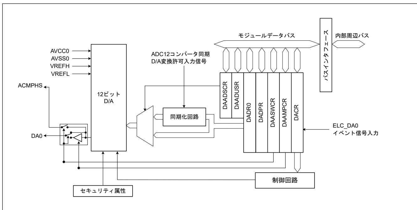
図 43.1 DAC12 のブロック図
