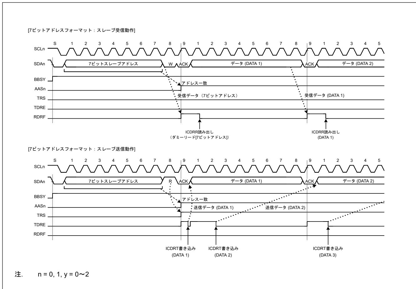
図 31.24 AASn フラグが 1 になるタイミング (7 ビットアドレスフォーマット選択時)
