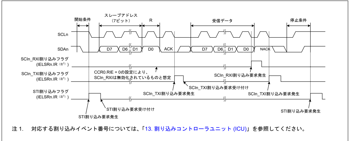
図 30.94 簡易 IIC モードにおけるマスタ受信の動作例 (7 ビットスレーブアドレス、送信割り込み、受信割り込み使用時) (ICR.IICINTM = 1)
