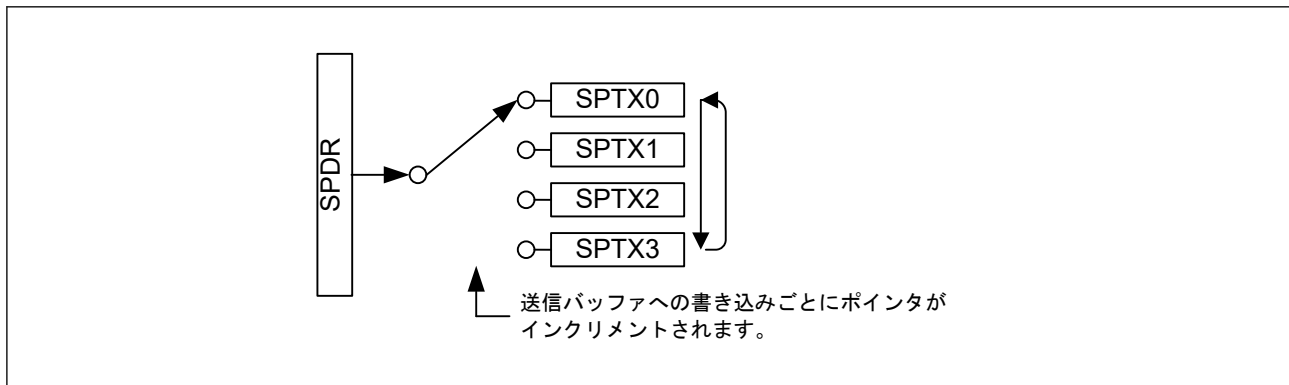
図 34.4 SPDR の構造（書き込み）
