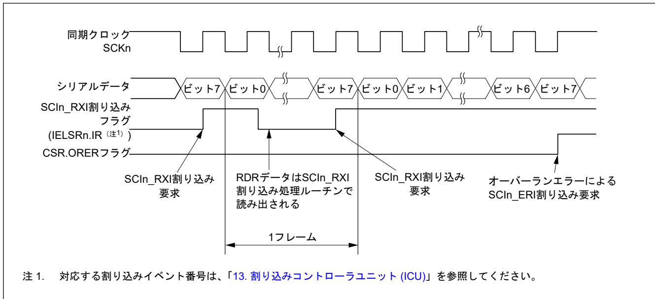
図 30.67 クロック同期式モードにおけるシリアル受信の動作例 (1) (RTS 機能を使用しない場合)
