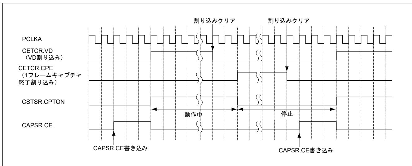
図 50.47 キャプチャ時の動作ステータス
