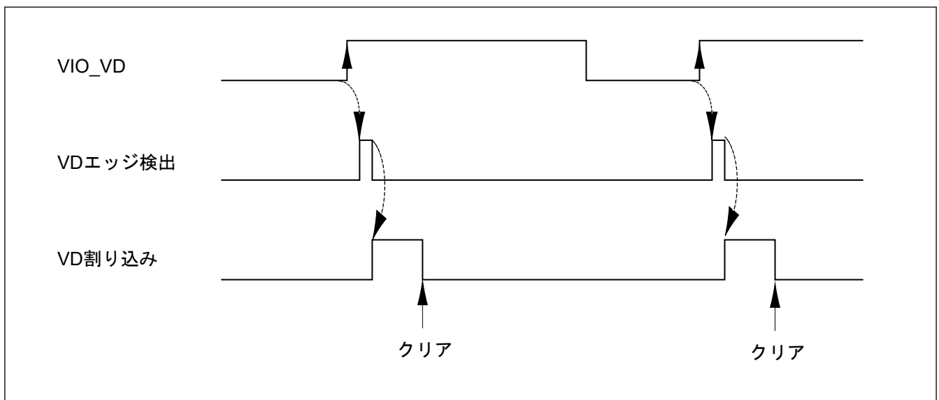
図 50.14 VD が正極性の場合の VIO_VD と VD 割り込みの関係(データイネーブル取り込みモードの場合)
