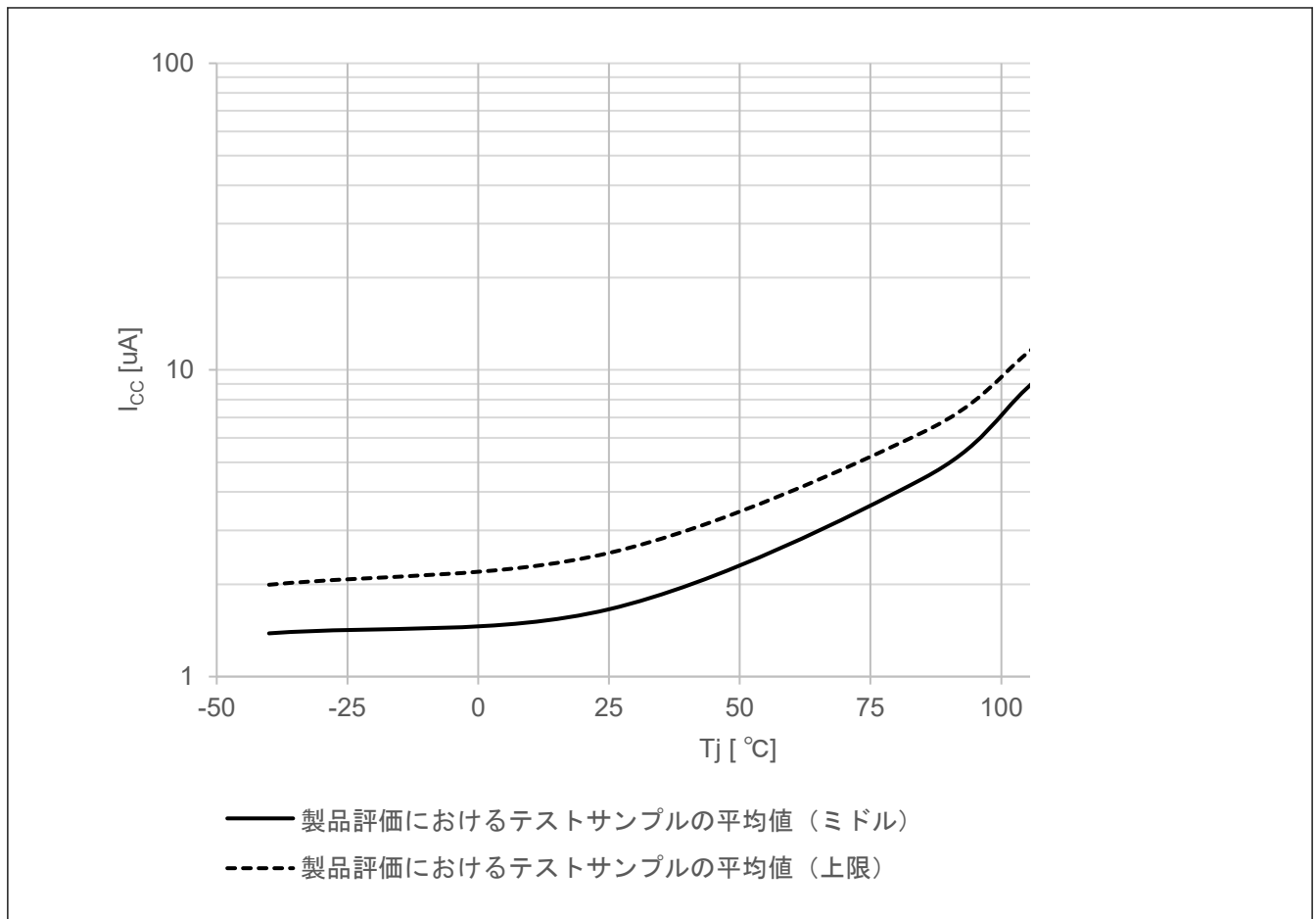
図 52.6 ディープソフトウェアスタンバイモード2における温度依存性 (参考データ)
