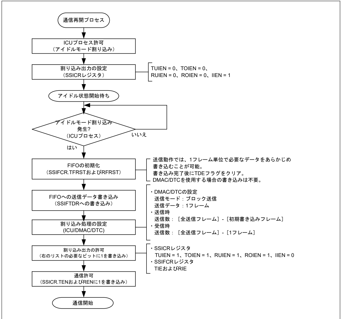
図 37.58 通信再開手順 (CPU 動作手順)
