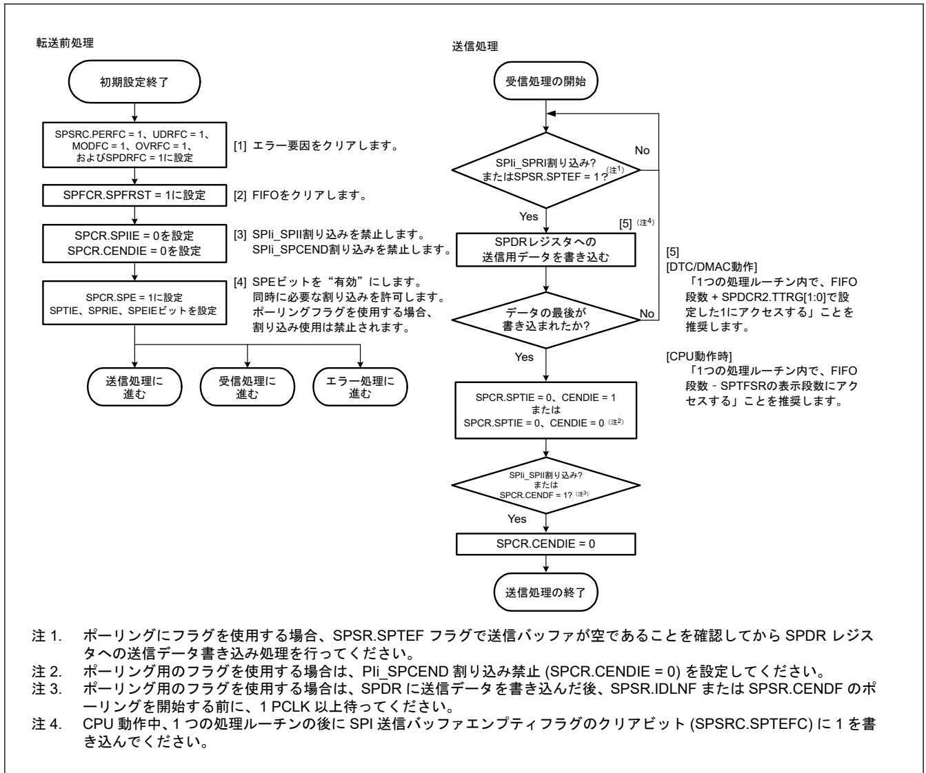
図 34.69 スレーブモードでの送信フロー
