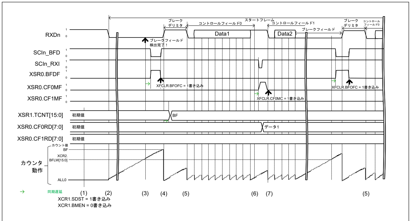
図 30.106 Control Field 1 の場合に Break Field を検出するスタートフレーム受信例 (PIB は未使用)
