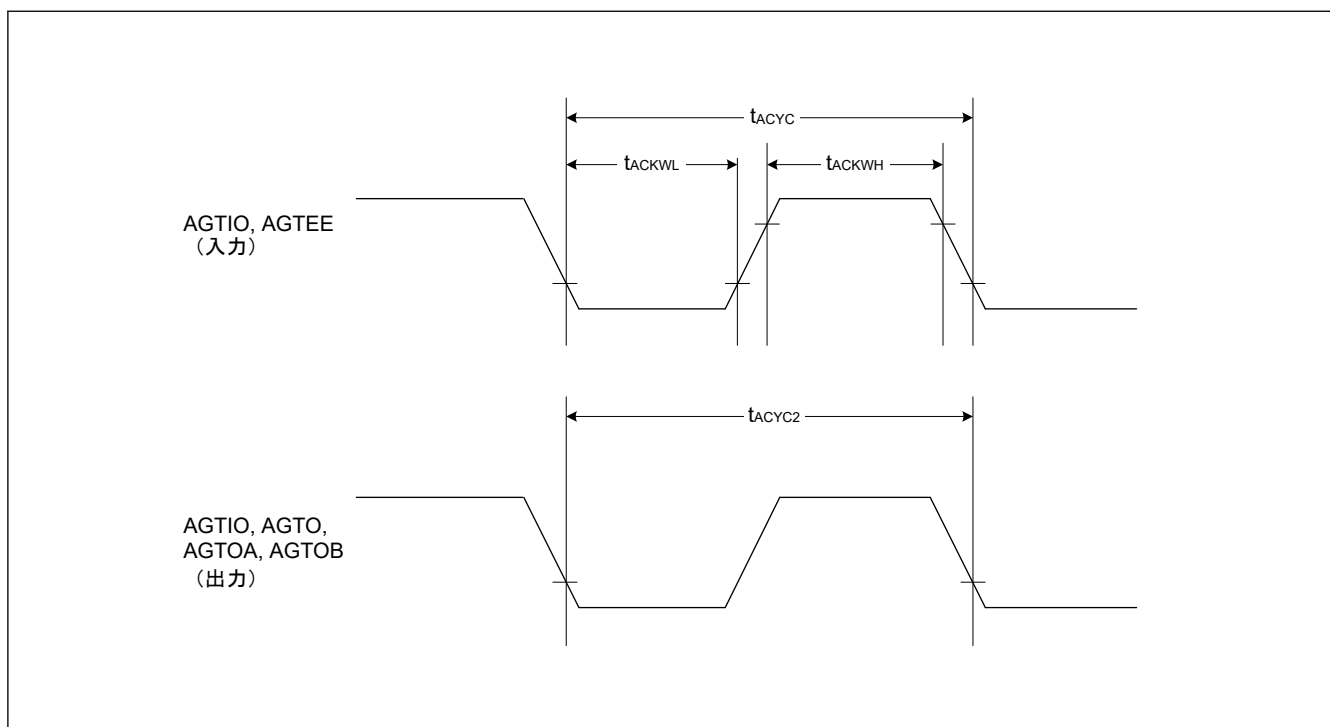
図 52.32 AGT 入出力タイミング
