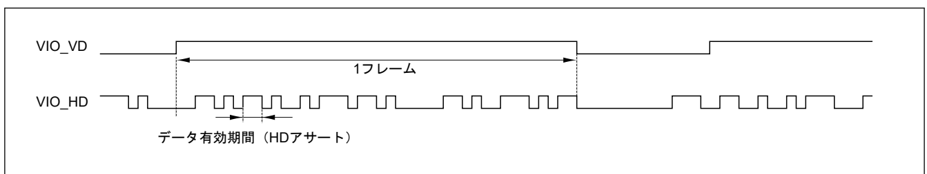
図 50.5 フレームのタイミング (データイネーブル取り込みの場合)
