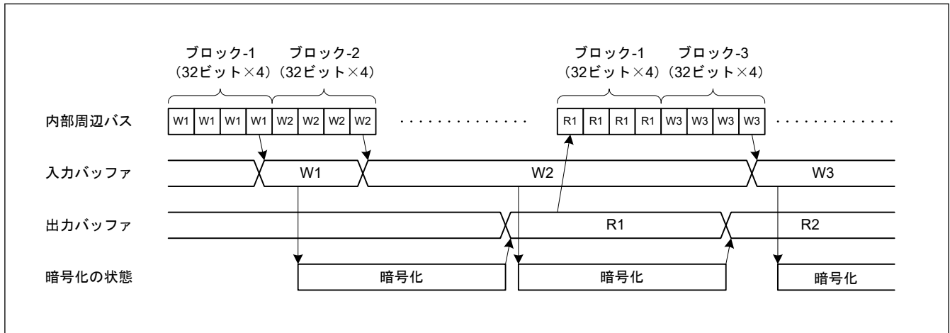
図 41.5 暗号／復号処理タイミング (AES)
