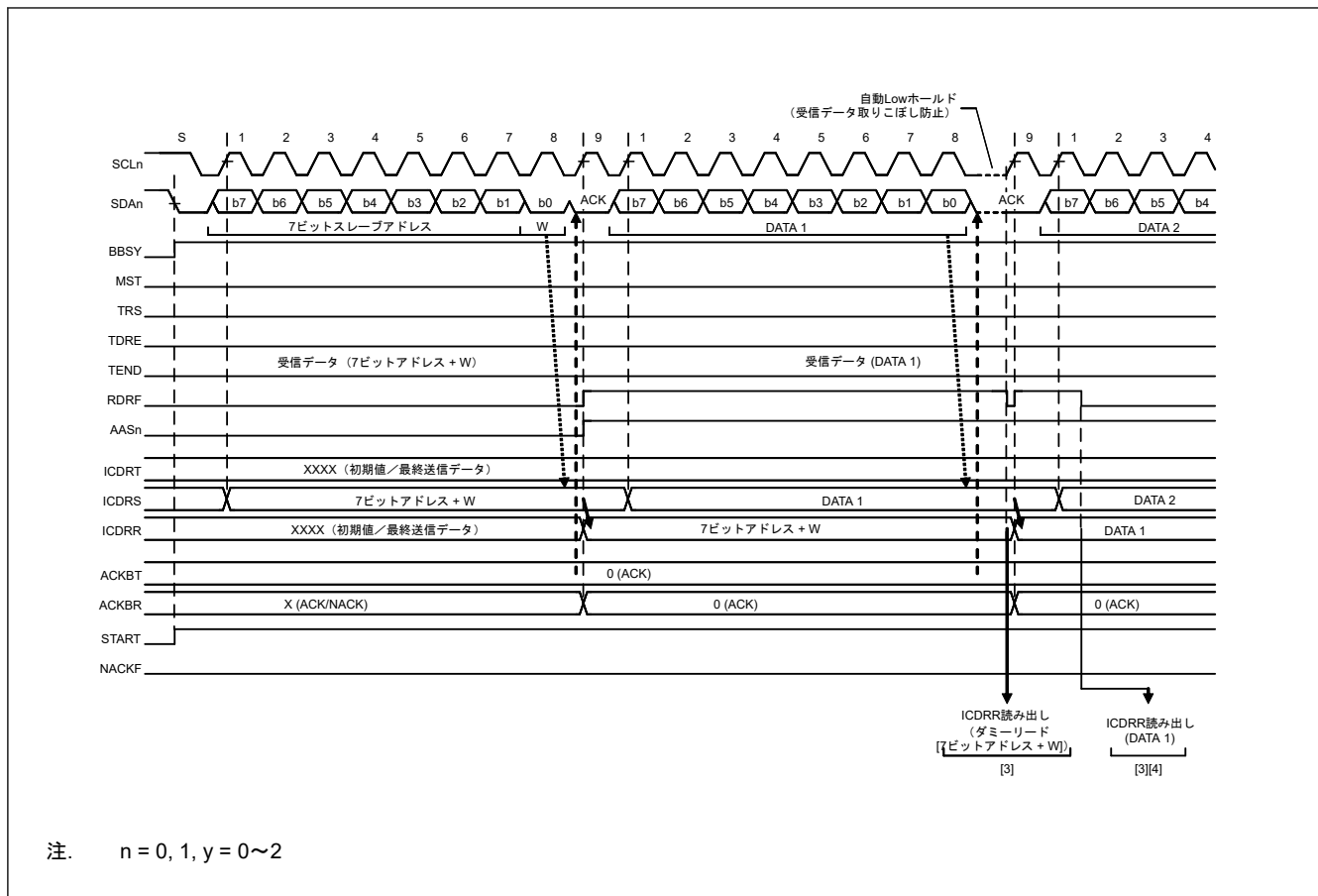
図 31.19 スレープ受信の動作タイミング (1) (7ビットアドレスフォーマットでRDRFS = 0の場合)
