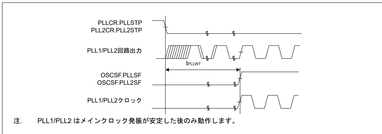
図 52.18 PLL1/PLL2 クロック発振開始タイミング
