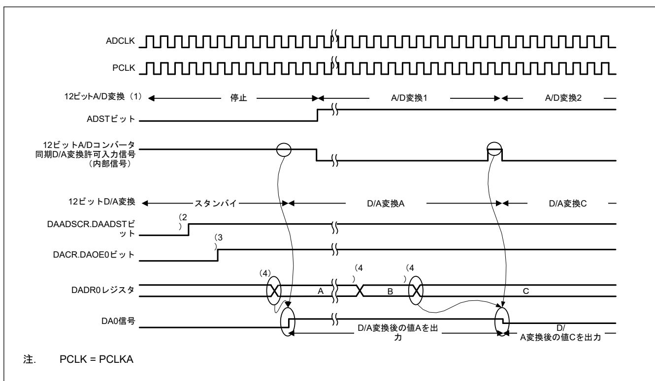
図 43.3 DAC12 を ADC12 (ユニット 1) に同期して変換する例
