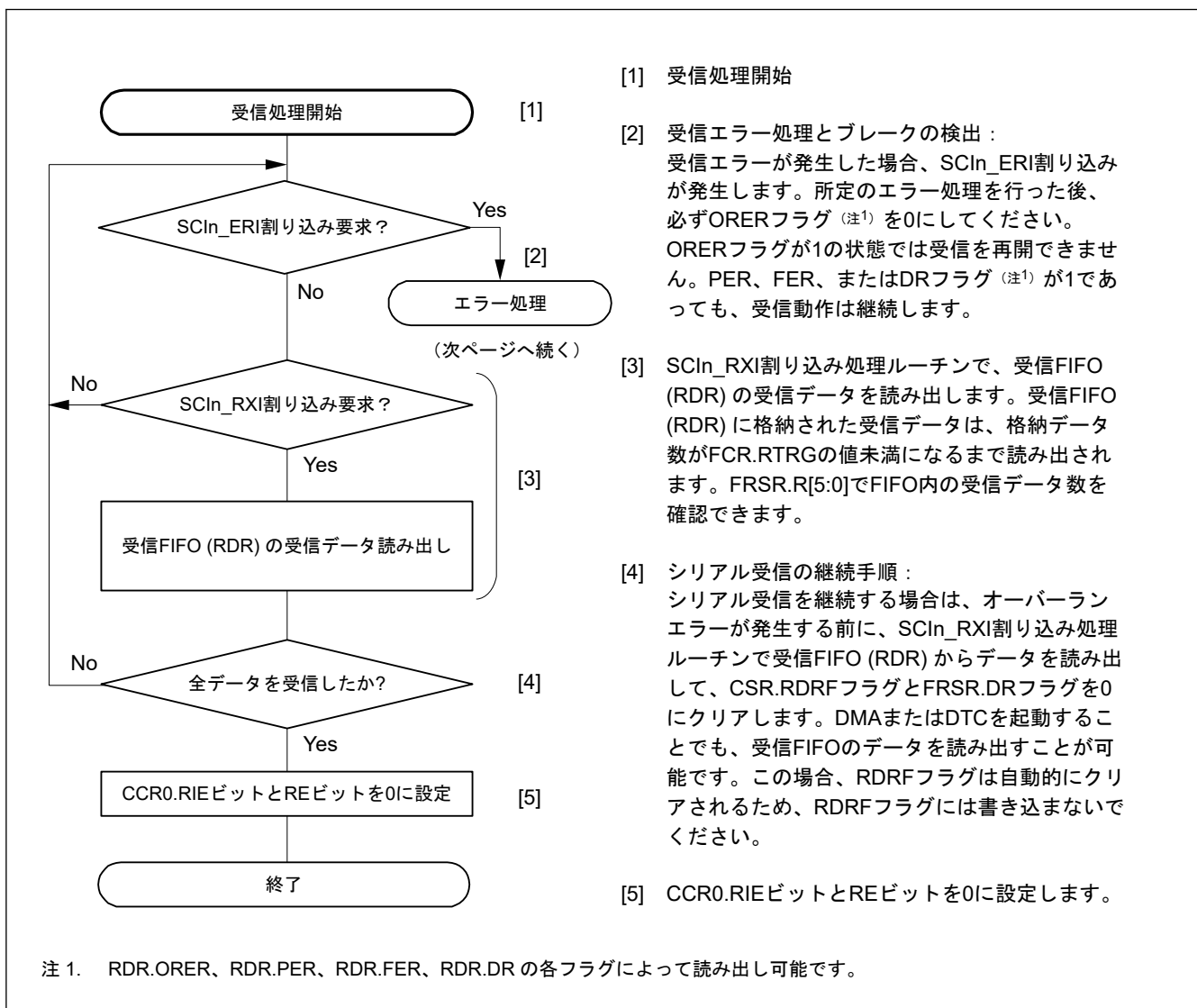
図 30.24 調歩同期式モードにおけるシリアル受信のフローチャート例 (FIFO 選択、アドレス一致検出有効時) (1)
