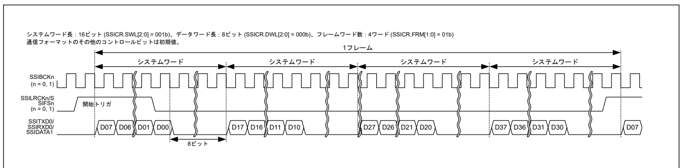
図 37.42 TDM フォーマット (パディングあり、システムワード長 > データワード長)
