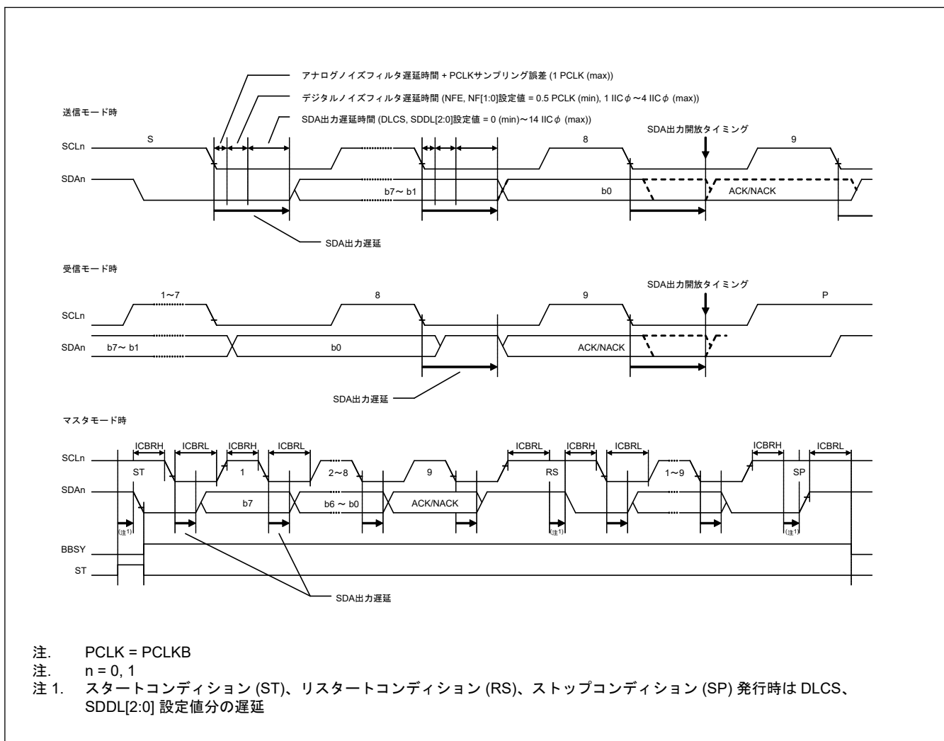
図 31.22 SDA 出力遅延機能
